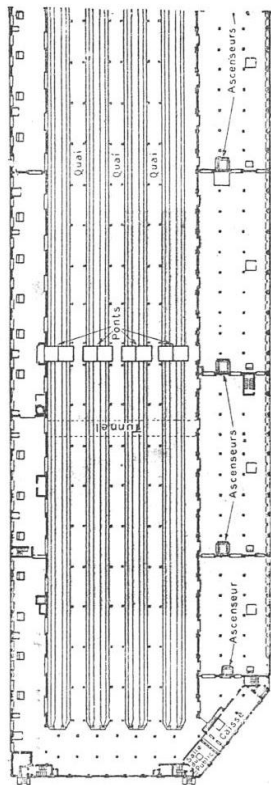
PLAN D'UNE GARE A MARCHANDISES COUVERTE A QUATRE VOIES
