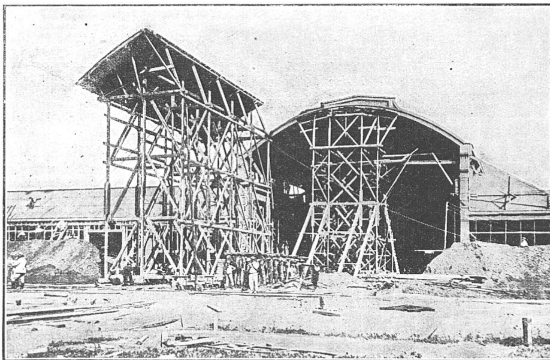
LA CONSTRUCTION DE LA TOITURE DE L'UN DES HALLS EN CIMENT ARMÉ
