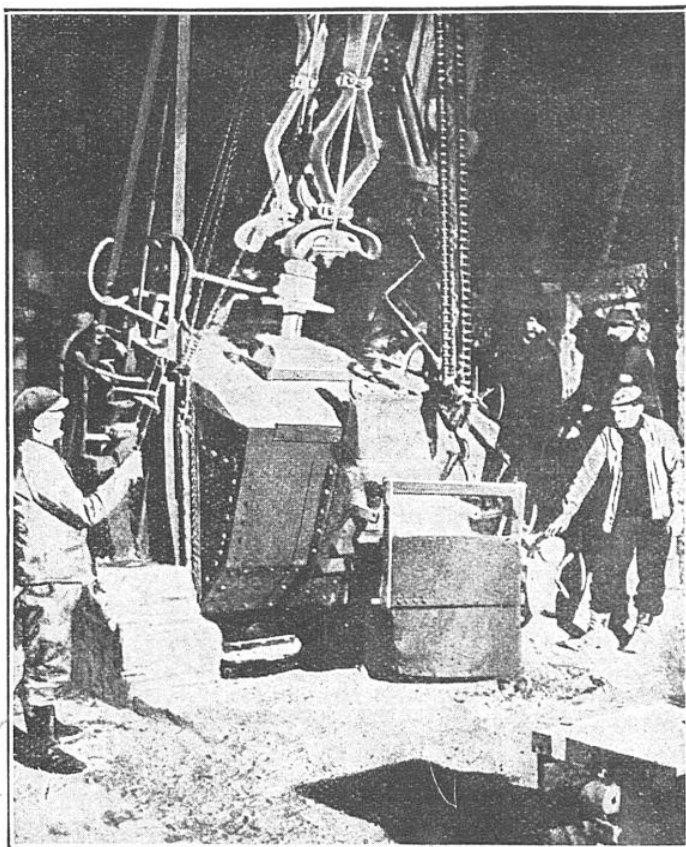
COULÉE DE FONTE SYNTHÉTIQUE POUR LA FABRICATION DES OBUS DE 400 MILLIMÈTRES
