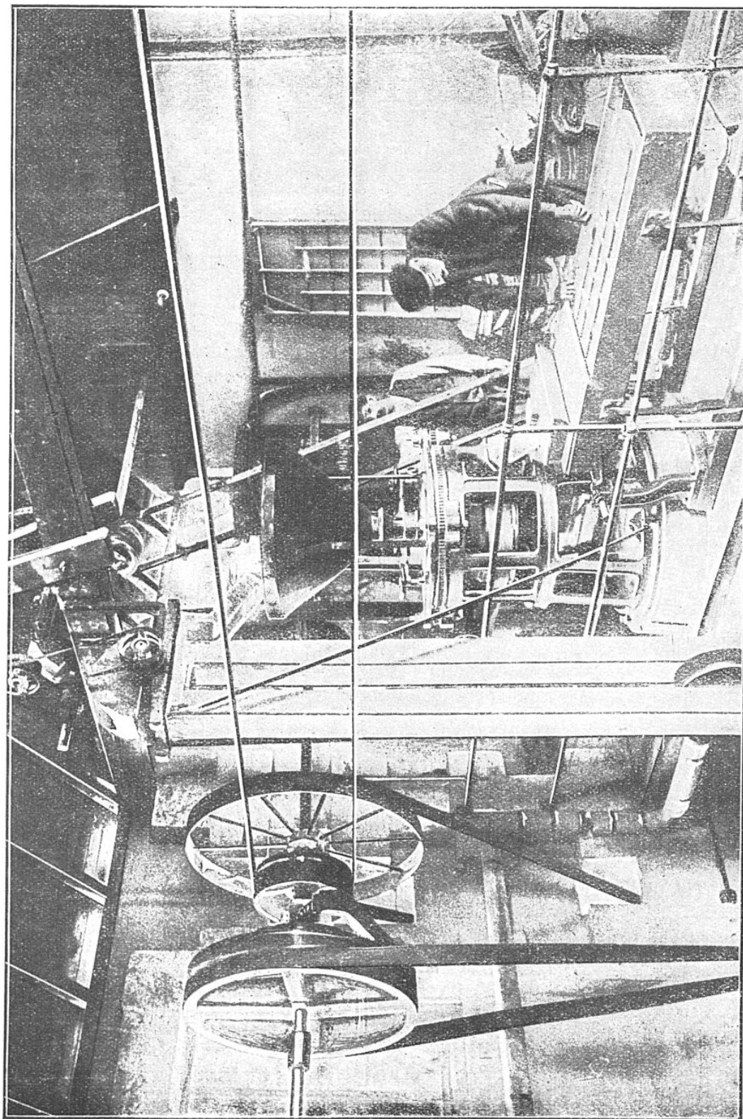
VUE GÉNÉRALE D'UNE INSTALLATION MÉCANIQUE POUR LA MOUTURE DE LA CASÉINE, DANS UNE GRANDE USINE DES CHARENTES.
