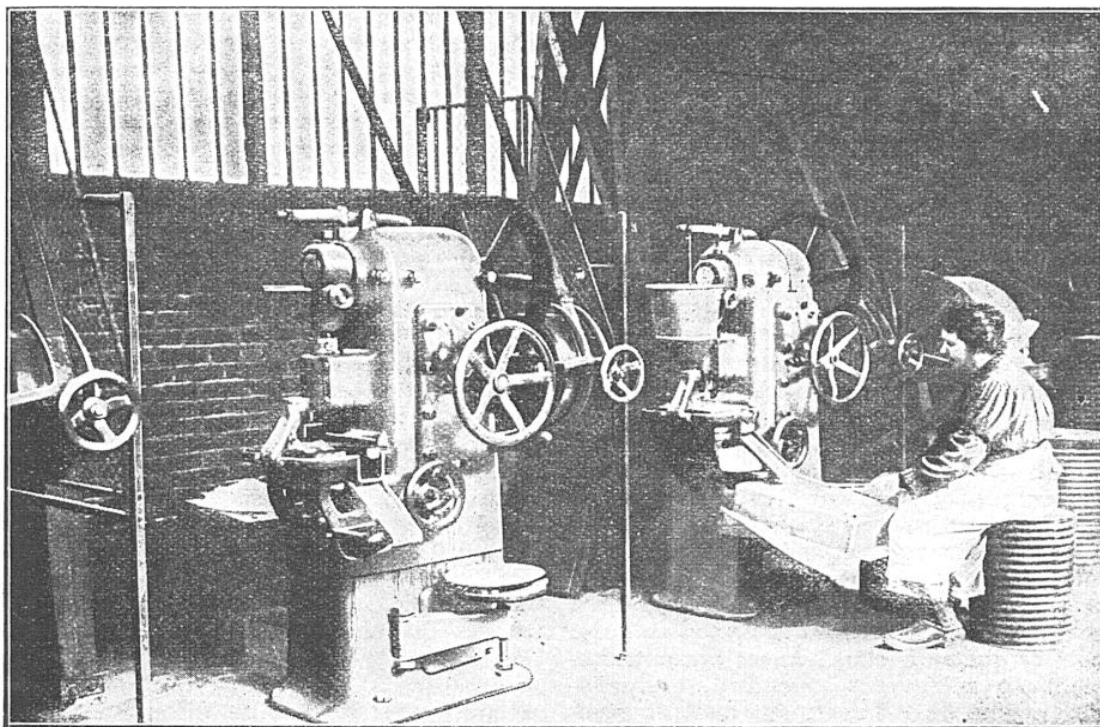
VUE PARTIELLE D'UN ATELIER DE PASTILLAGE DE SACCHARINATE DE SOUDE
