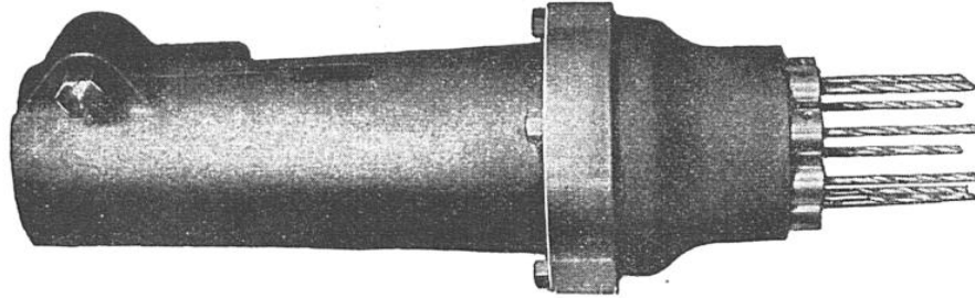
MANDRIN A HUIT FORETS SYMÉTRIQUES MAIS NON ORIENTABLES
