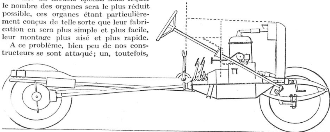
COUPE SCHÉMATIQUE DU CHÂSSIS, MONTRANT LA DISPOSITION DES ORGANES
