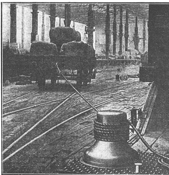
CABESTAN ÉLECTRIQUE EN ACTION
