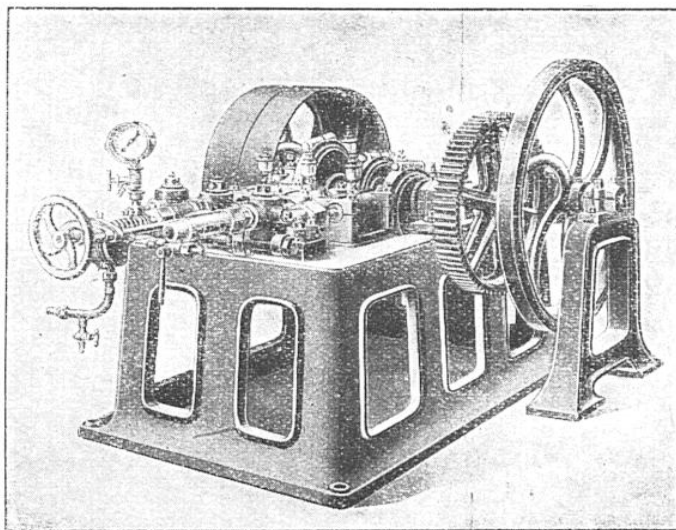
APPAREIL HOMOGÉNÉISATEUR GAULIN
