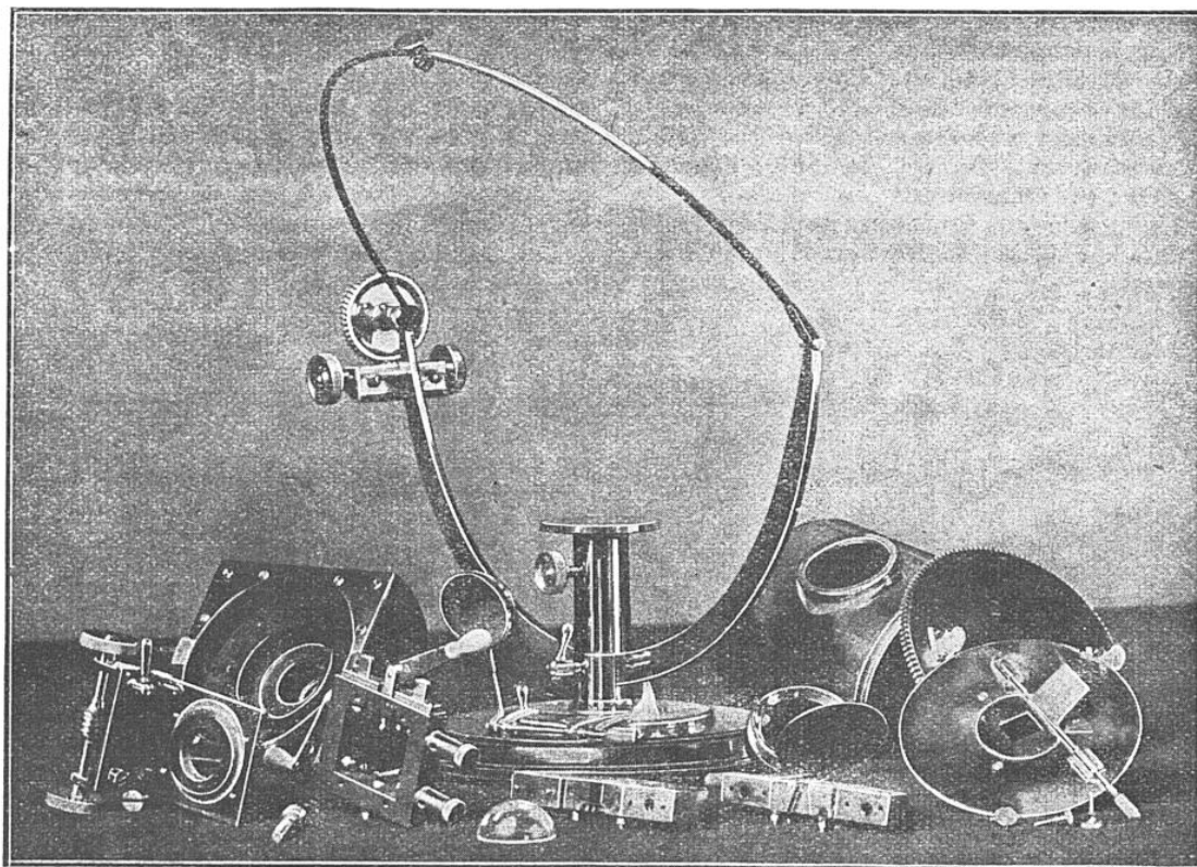
LES DIVERSES PIÈCES (DÉMONTÉES) DU PYRANOMÈTRE ABBOTT-ALDRICH
