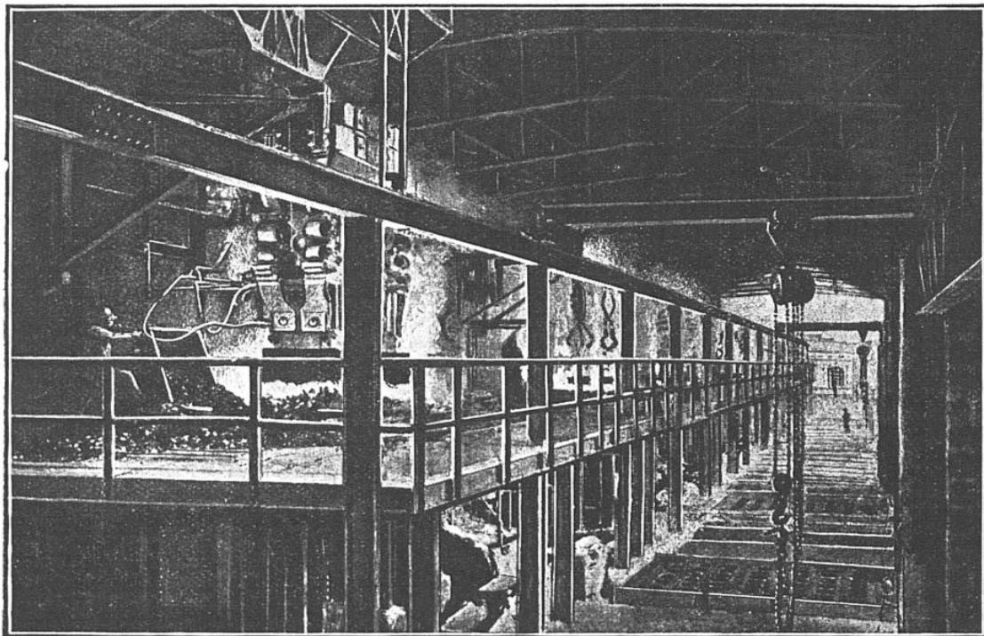
AUTRE HALL DE FOURS ÉLECTRIQUES INSTALLÉS AUX USINES DE LIVET (ISÈRE) On voit ici, rangés en une batterie, quatre fours de 2.000 kilowatts et un four de 2.500 kilowatts.
