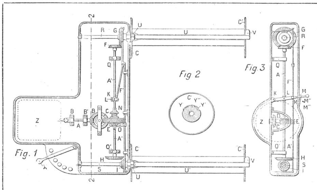
DÉTAIL DES ORGANES MÉCANIQUES QUI COMPOSENT L'APPAREIL DE M. U. BERTRAND
