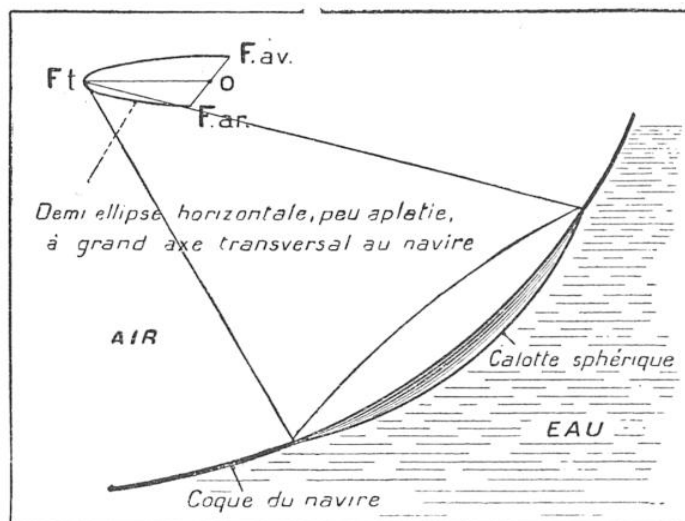
Ft, est le foyer pour la direction transversale; F. av. et F. ar., sont les foyers pour les directions de l'avant et de l'arrière respectivement; il y a donc un foyer caractéristique pour chaque relèvement de la source sonore (appareil Walser).
