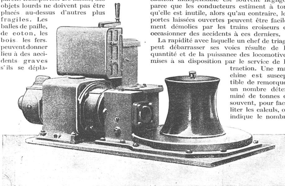
CABESTAN ÉLECTRIQUE AVEC MÉCANISME DÉCOUVERT REMPLAÇANT LES CHEVAUX
