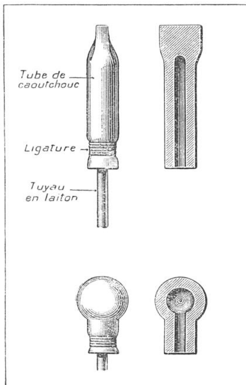
LE TUBE « C » DES AMÉRICAINS
