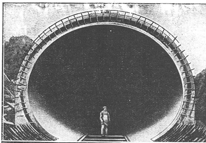
CETTE CANALISATION EST DE SECTION OVALE ET NON RONDE COMME L'AUTRE; ELLE EST ENTIÈREMENT EN BÉTON ARMÉ
