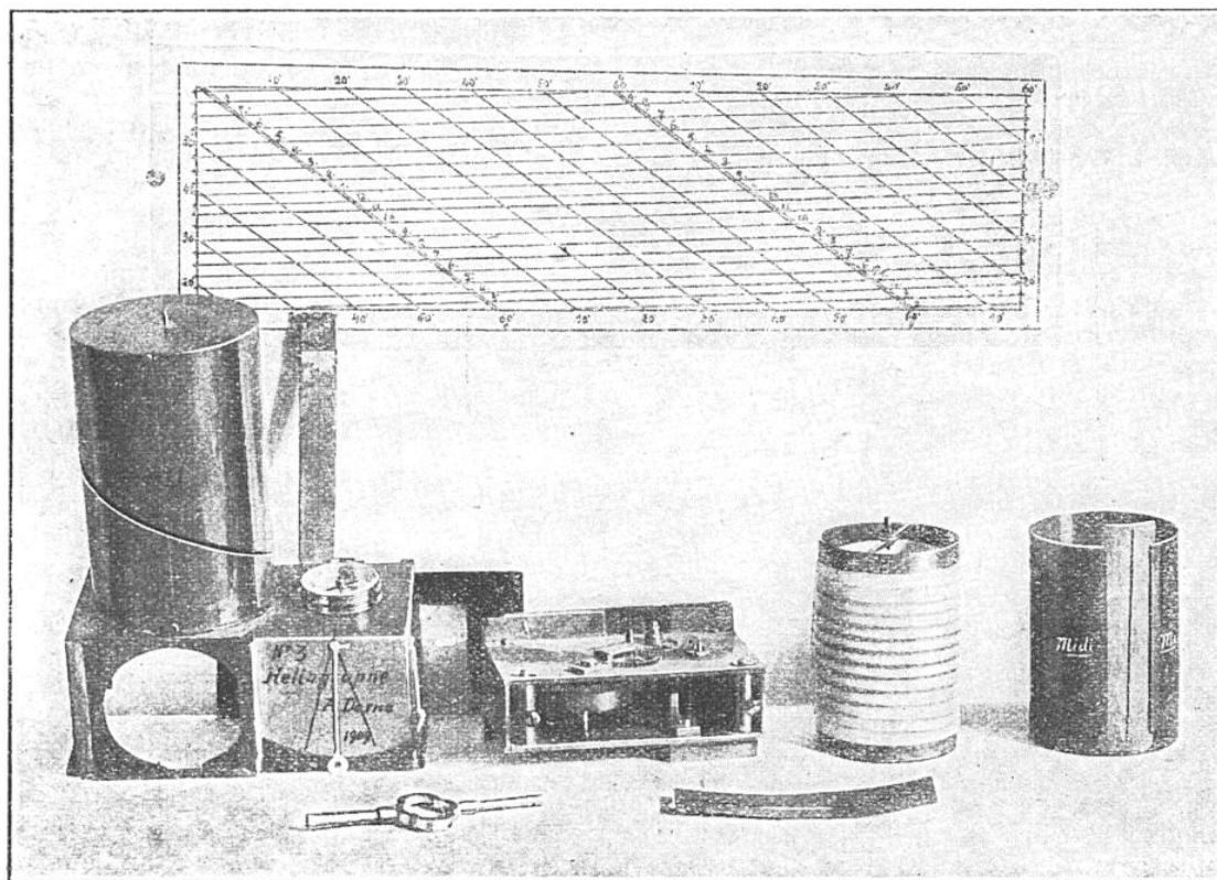
LES DIFFÉRENTES PARTIES DE L'HÉLIOGRAPHE PHOTOGRAPHIQUE DOSNE, DÉMONTÉ
