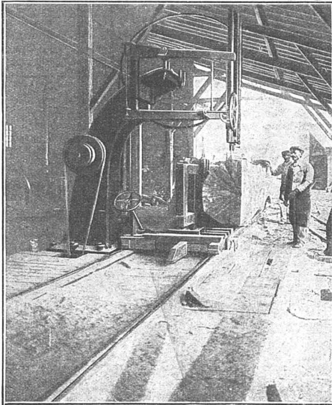
LES BOIS EN GRUME DÉBITÉS MÉCANIQUEMENT
