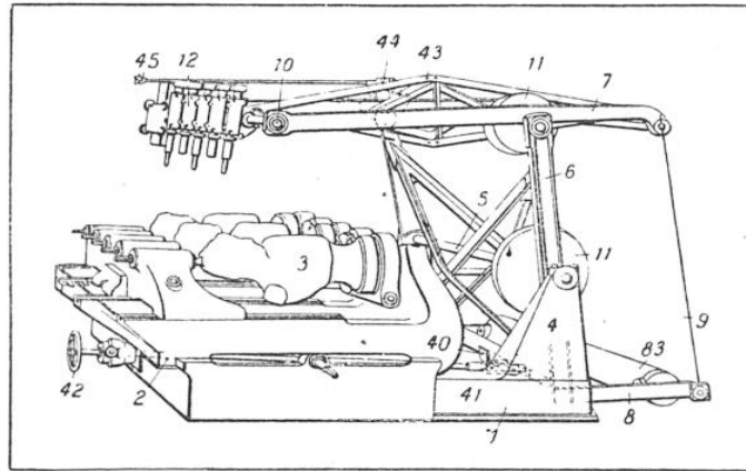
MACHINE A REPRODUCTIONS MULTIPLES DE M. PETERS (VUE D'ENSEMBLE)
