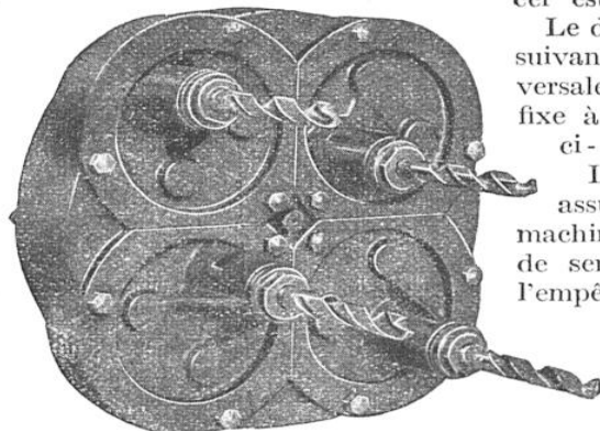
MANDRIN A QUATRE MÈCHES ORIENTABLES PAR RAPPORT AU CENTRE DU SYSTÈME
