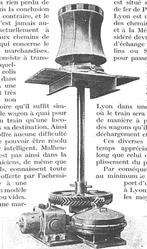
CABESTAN A MÉCANISME ÉLECTRIQUE SOUTERRAIN POUR HALAGE DE PÉNICHES DANS UNE GARE D'EAU SITUÉE LE LONG D'UN CANAL
