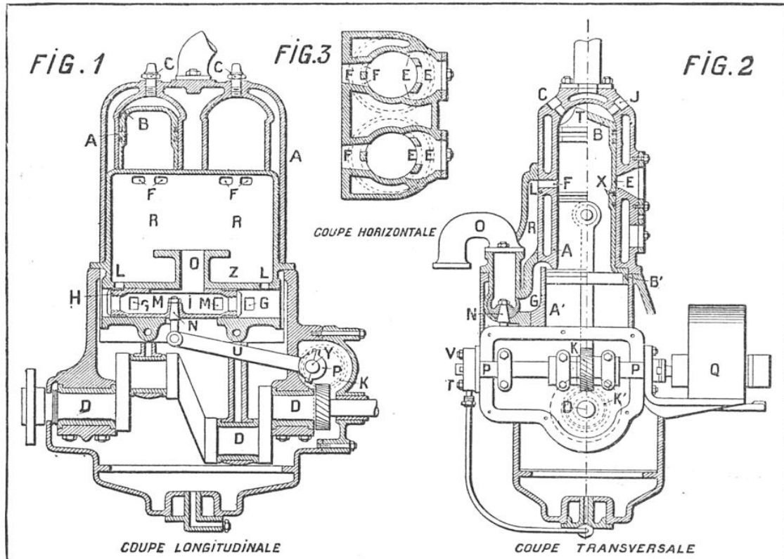
COUPES D'UN MOTEUR D'AUTO A DEUX TEMPS, SANS SOUPAPE
