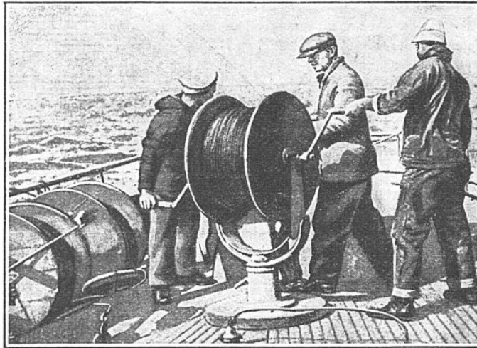
CERTAINS APPAREILS AMÉRICAINS ÉTAIENT REMORQUÉS AU BOUT D'UNE LIGNE ENROULÉE SUR UN TREUIL, AFIN DE LES ISOLER DES BRUITS DU NAVIRE
