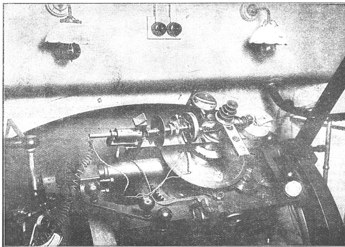
PHOTOMÈTRE STELLAIRE NORDMANN MONTÉ POUR UNE OBSERVATION
