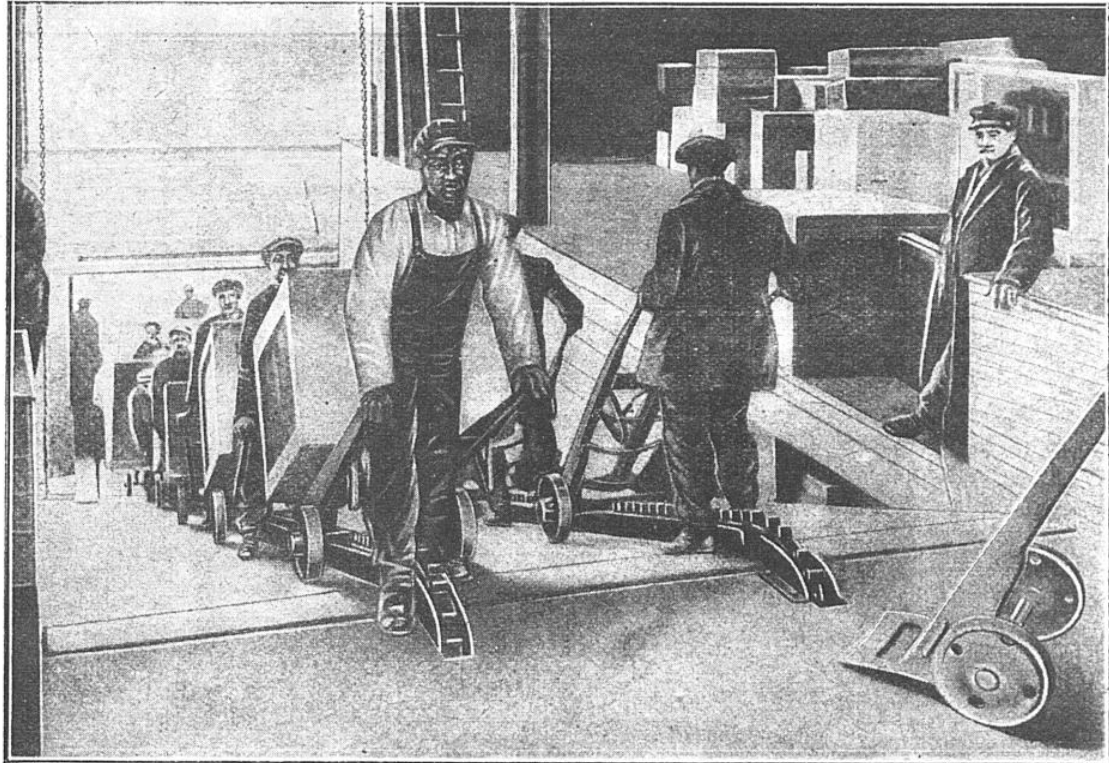
BATTERIE D'ÉLÉVATEURS A CHARIOTS DANS UNE GARE DE TRANSIT AMÉRICAINE
