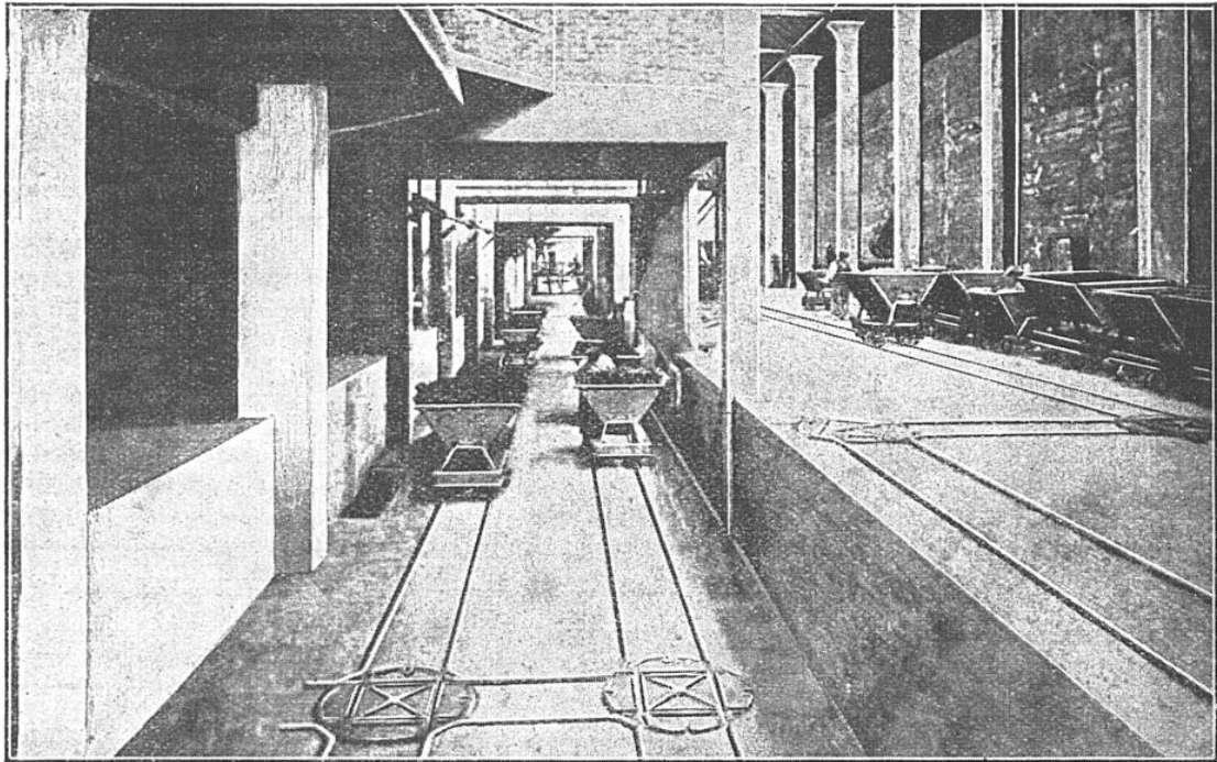
VOIES DE REPRISE DES LITS DE FUSION A LA FONDERIE NATIONALE DE NANTERRE
