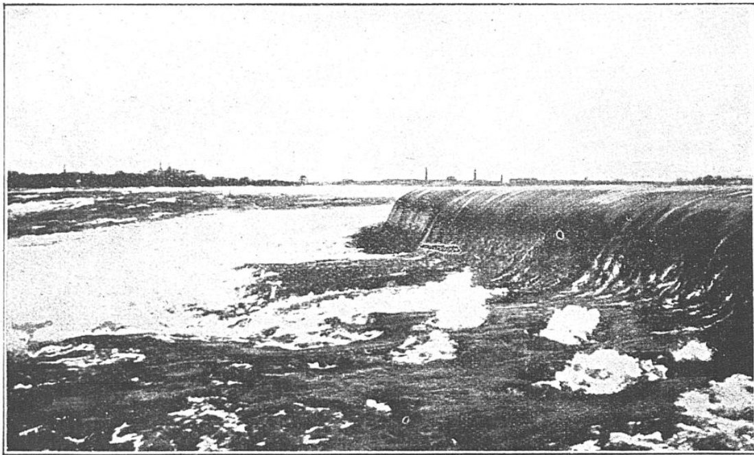
DIGUE SUBMERGÉE FAISANT PARTIE DES OUVRAGES SITUÉS EN AMONT DES CHUTES L'excès de l'eau qui est nécessaire à l'alimentation de la centrale, fait retour aux rapides supérieurs en passant par-dessus cette digue ; il entraîne avec lui glaçons et débris minéraux.
