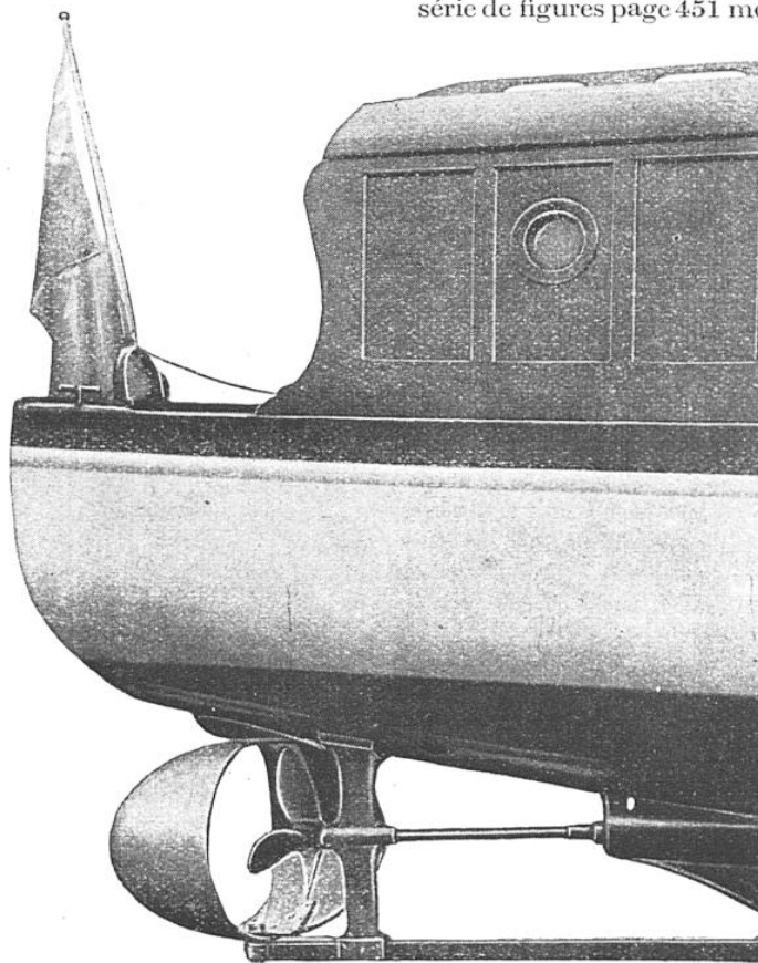
DISPOSITION DE L'ÉTAMBOT, DE L'ARBRE PORTE-HÉLICE ET DU GOUVERNAIL KITCHEN DANS UNE EMBARCATIION PONTÉE, A MOTEUR
