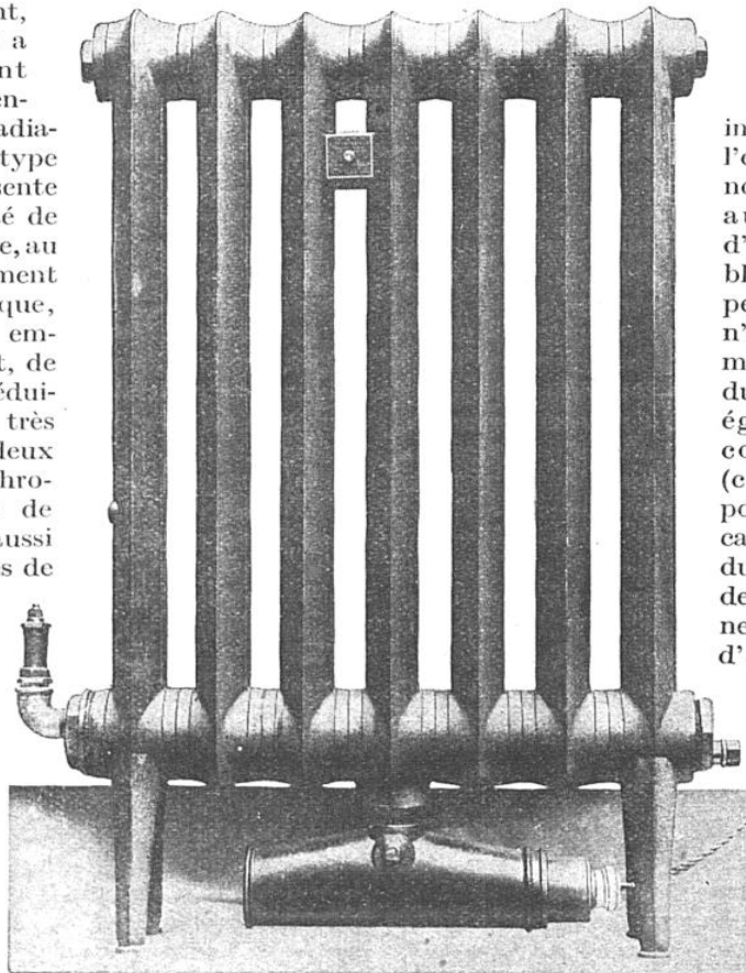
LE RADIATEUR AVEC SON FOYER ÉLECTRIQUE
