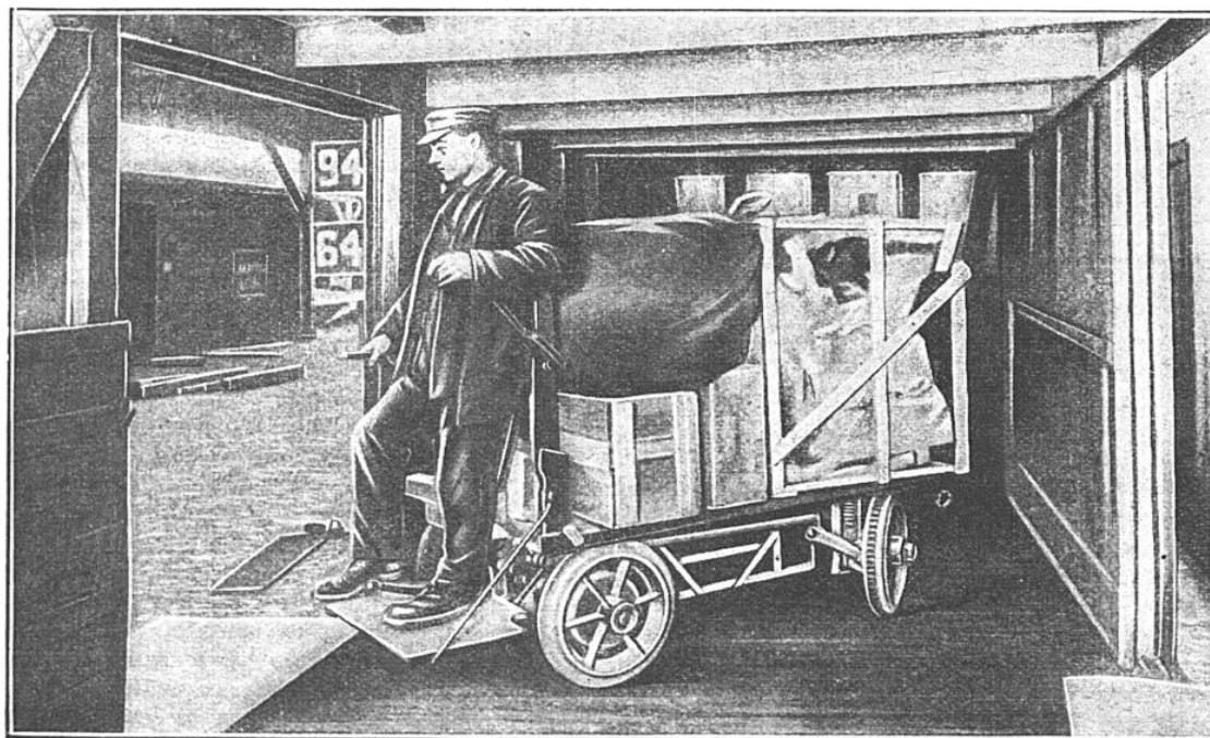
CHARIOT ÉLECTRIQUE VIDANT UN WAGON DE SON CHARGEMENT C'est grâce à l'emploi de quais surélevés qu'on peut utiliser ces véhicules silencieux et rapides.
