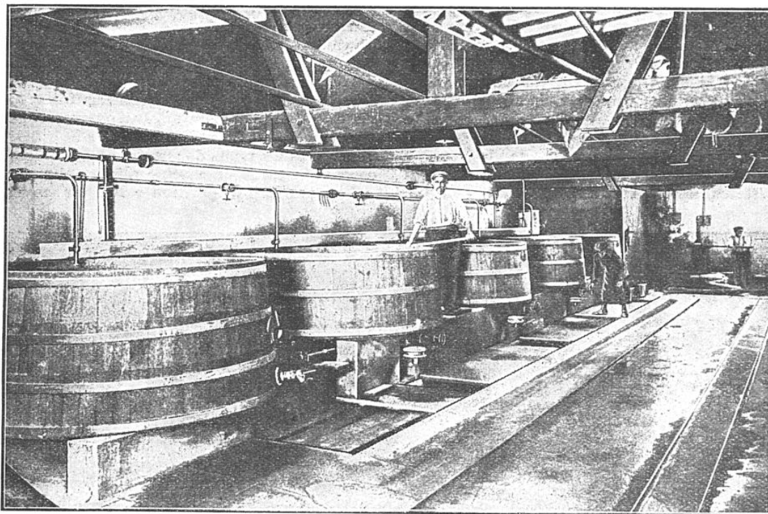
BATTERIE DE CUVES A PRÉCIPITATION DU LAIT APRÈS ÉCRÉMAGE
