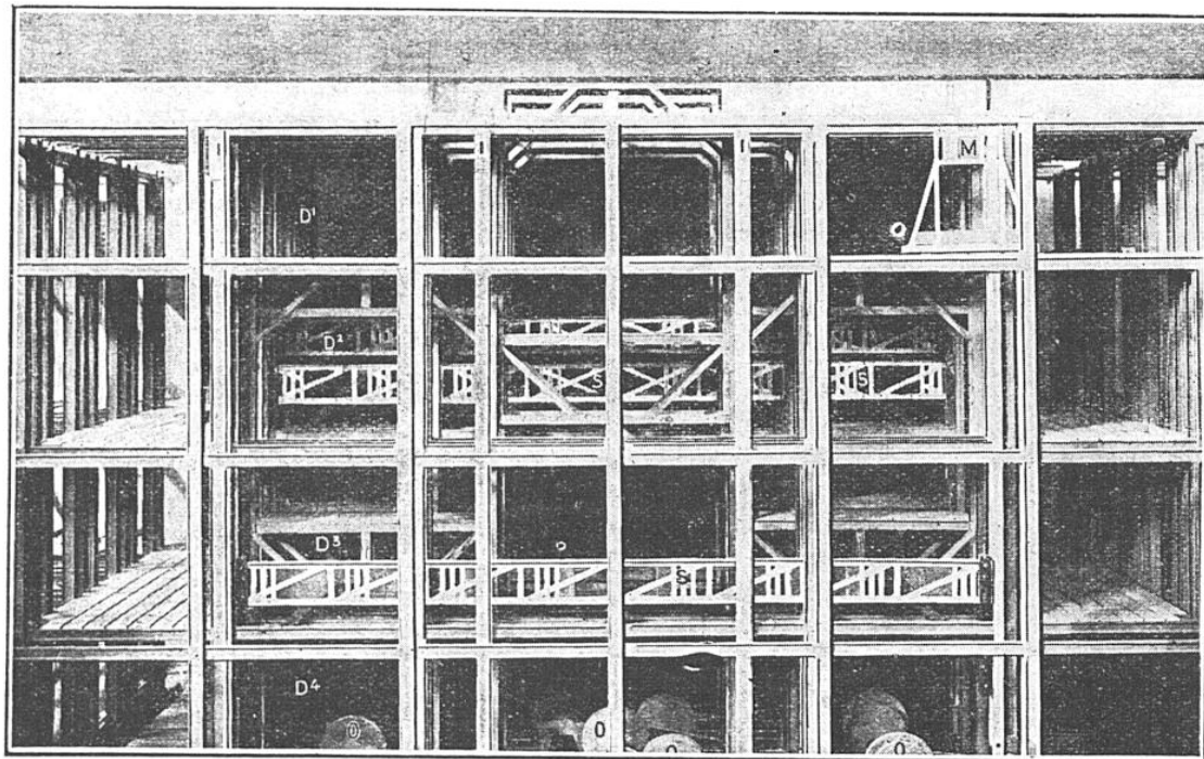
DISPOSITION GÉNÉRALE DES DESSOUS D'UN THÉÂTRE ET LEUR MACHINERIE
