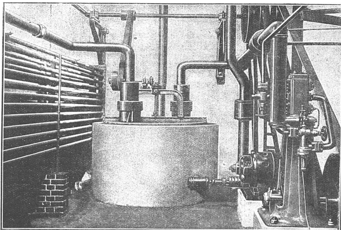
LA MACHINE FRIGORIFIQUE SPÉCIALE AVEC SA TUYAUTERIE
