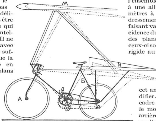
COUPE SCHÉMATIQUE DE L'AVIETTE POULAIN
