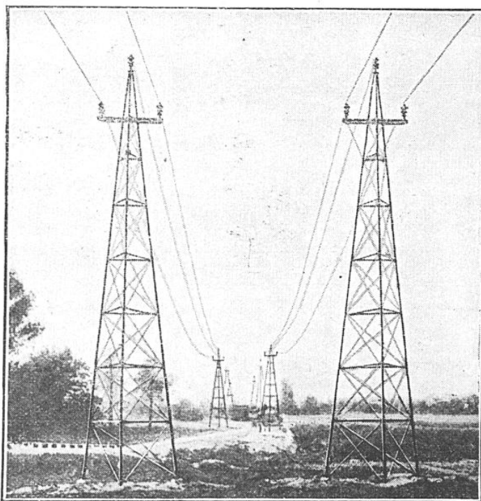
PYLONES EN ACIER SUPPORTANT LES LIGNES DE TRANSPORT DE FORCE A 60.000 VOLTS
