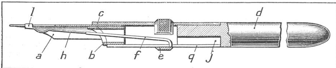
SUR LE PORTE-PLUME ORDINAIRE, LE SERRE-BEC FORME UNE RÉSERVE D'ENCRE
