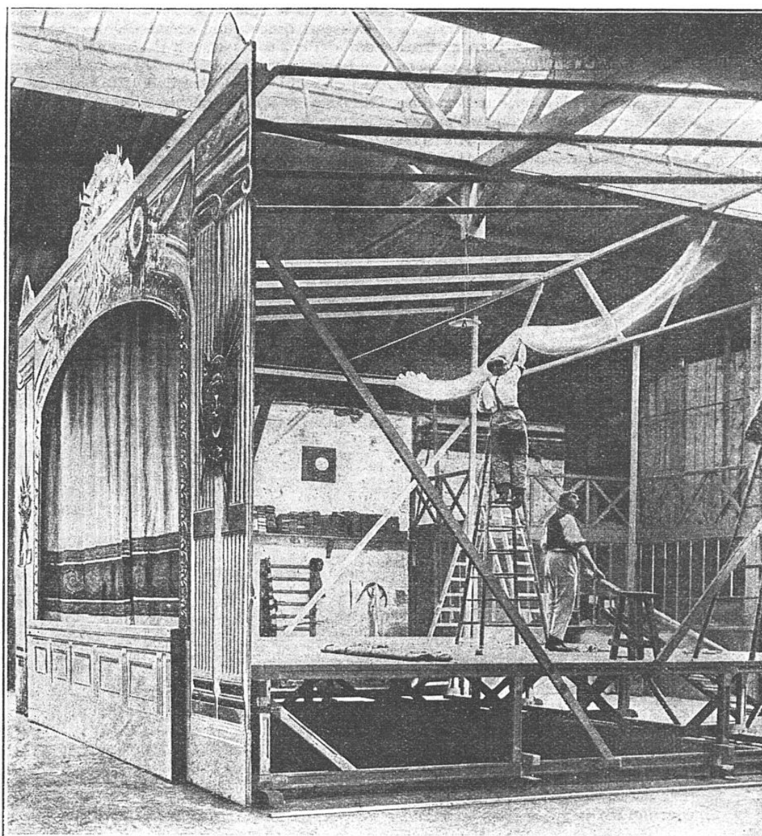
LA FAÇADE DE LA SCÈNE DÉMONTABLE EST DRESSÉE, LES MACHINISTES SONT MAINTENANT OCCUPÉS A PLACER LES FRISES ET A DISPOSER LE PLAFOND
