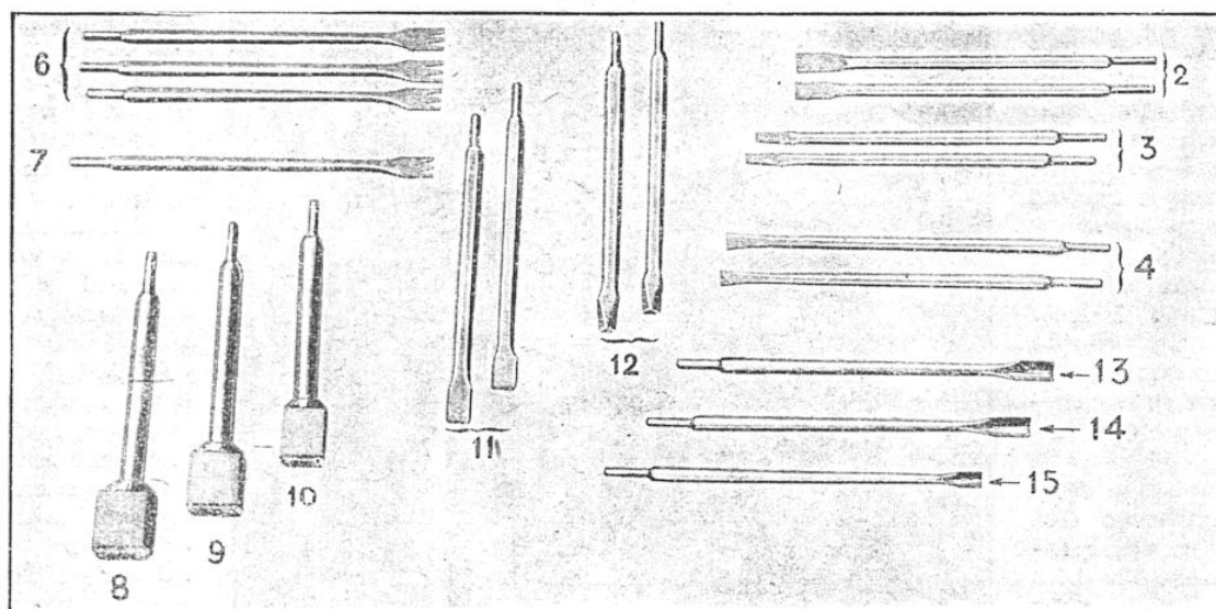
FORMES DIVERSES D'OUTILS A SCULPTER POUR MARTEAUX PNEUMATIQUES
