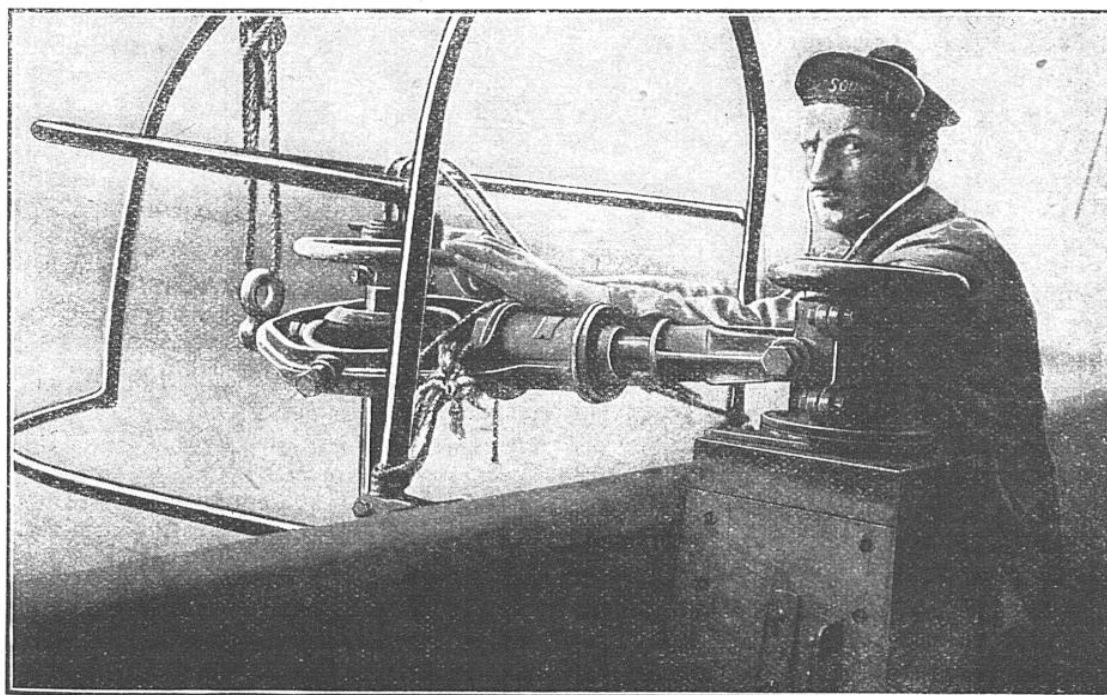
TUBE « C » AMÉRICAIN, INSTALLÉ SUR UN CHASSEUR DE SOUS-MARINS FRANÇAIS
