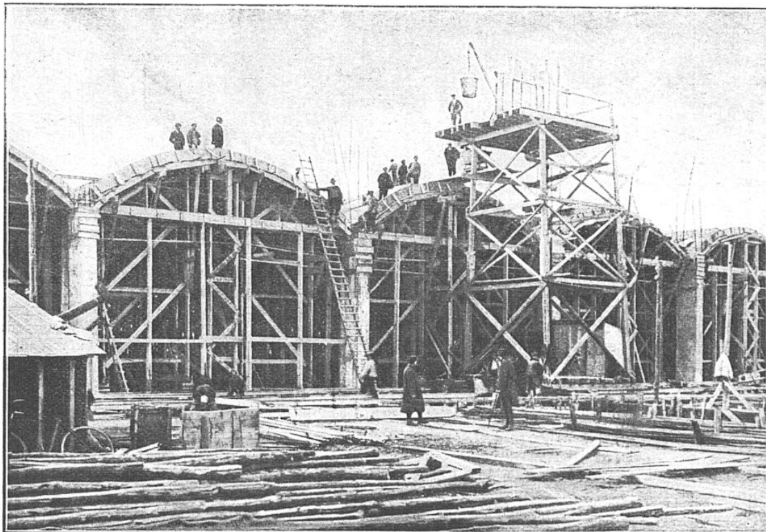
SÉRIE DE TRAVÉES PARALLÈLES EN CIMENT ARMÉ, EN COURS DE CONSTRUCTION
