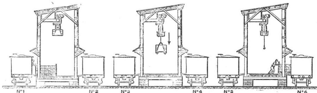
COUPE D'UNE INSTALLATION DE CHARGEMENT RAPIDE POUR COLIS DIVERS
