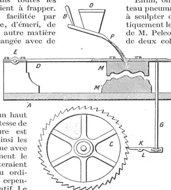
APPAREIL DE M. MOREAU POUR SCULPTER LES BAS-RELIEFS
