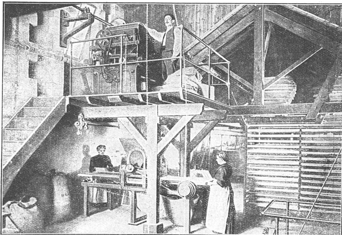
VUE GÉNÉRALE D'UNE INSTALLATION DE CHARGEMENT DE LA CAILLEBOTTE SUR LES CIAIES DE SÉCHAGE, POUR LA FABRICATION DE LA CASÉINE
