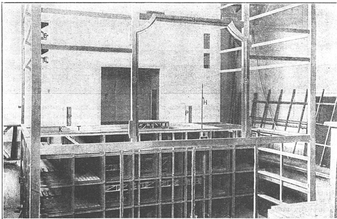
MAQUETTE EN COURS DE CONSTRUCTION DE LA SCÈNE D'UN GRAND THÉÂTRE B B B, cadre représentant la baie de la scène que ferme le rideau ; T, plancher mobile, trappes ; K, costières, H, mât mobile ; P P, portes de dégagement ; E E, escaliers de dégagement ; F, fond de la scène, lointain
