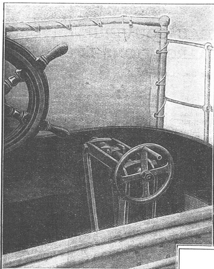
POSTE DU PILOTE DANS UNE EMBARCATION MUNIE DU GOUVERNAIL KITCHEN.
