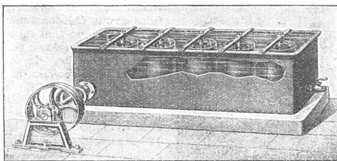
BAC A TOPETTES TOURNANTES
