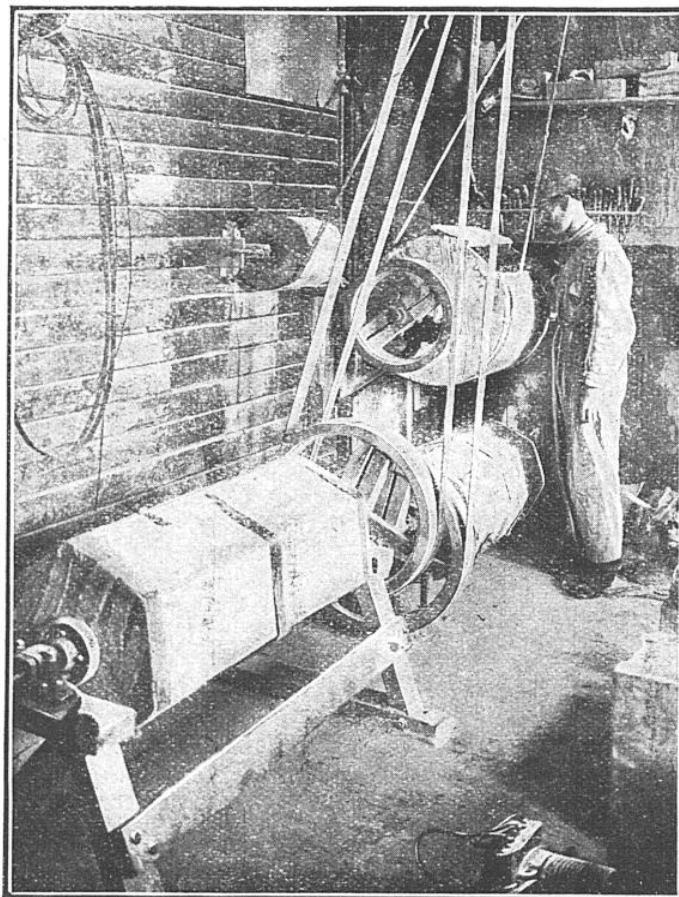
POLISSAGE DES OBJETS FABRIQUÉS AVEC L'OMNILITH
