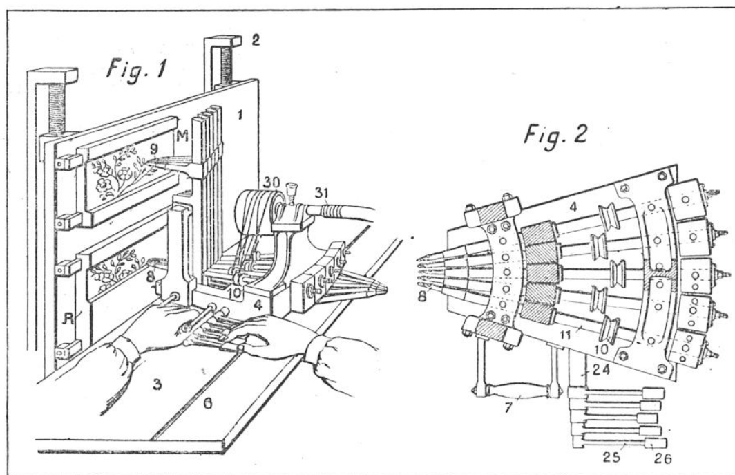
MACHINE A FRAISES MULTIPLES CONSTRUITE PAR M. SELMERSHEIM
