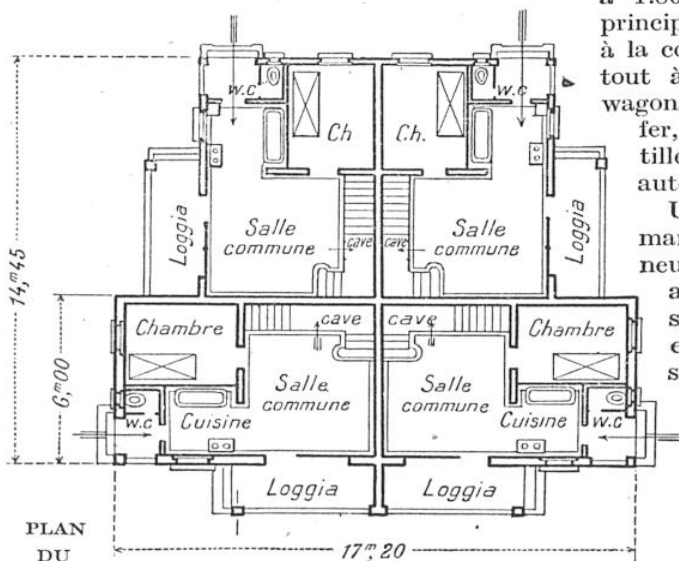
PLAN DU REZ-DE-CHAUSSÉE D'UN PAVILLON A QUATRE LOGEMENTS Les murs intérieurs en croix isolent complètement les locataires les uns des autres, ce qui écarte les promiscuités gênantes.
