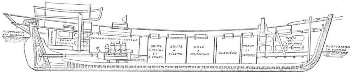
COUPE LONGITUDINALE D'UN HARANGUIER EN BOIS TYPE FÉCAMP
