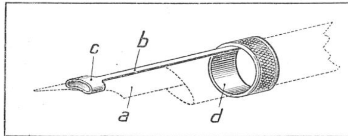
LE DISPOSITIF ADAPTÉ AU PORTE-PLUME RÉSERVOIR
