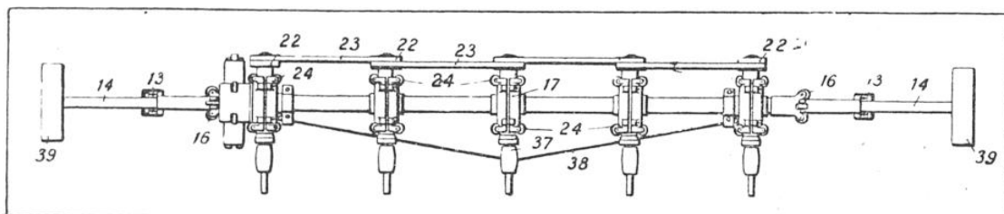
DÉTAIL DE LA MACHINE PETERS DESTINÉE AUX REPRODUCTIONS MULTIPLES
