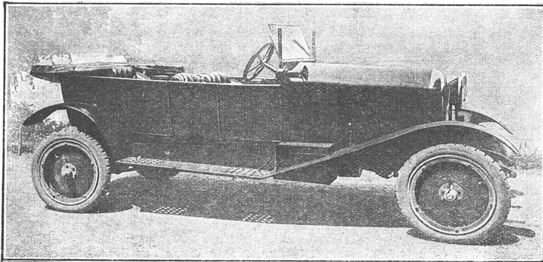
TYPE DE VOITURE, CAPOTE REPLIÉE, MONTRANT LE MODE DE CONSTRUCTION MÉTALLIQUE DE LA CARROSSERIE, DES ROUES, DES MARCHEPIEDS, DES AILES ET DES PHARES
