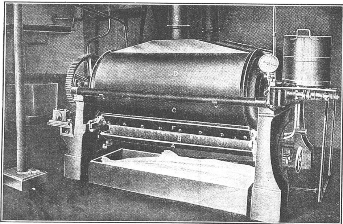
APPAREIL MIGNOT-PLUMÉY POUR LA FABRICATION DU LAIT EN POUDRE
