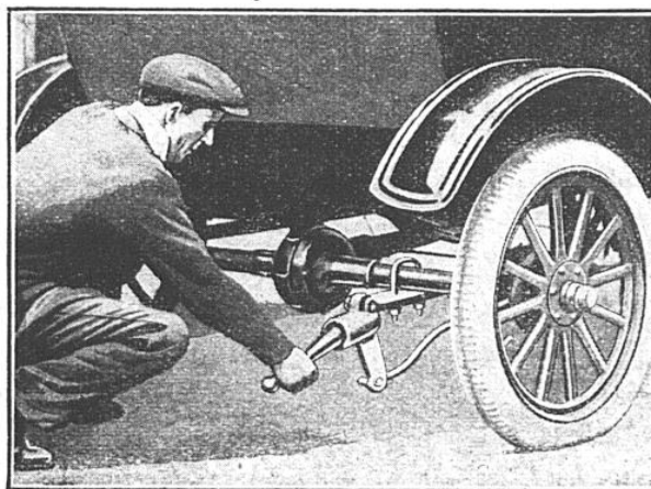
LA MARCHE DE LA VOITURE EST COMMANDÉE DE L'ARRIÈRE PAR LE CONDUCTEUR
