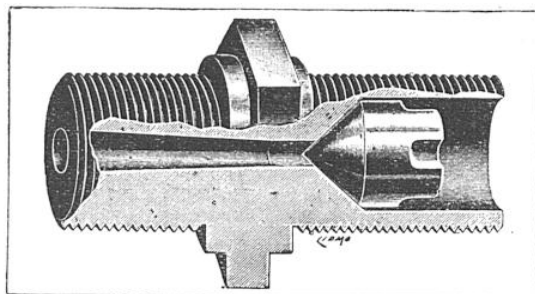
COUPE DU DISPOSITIF HOMOGENEISANT
