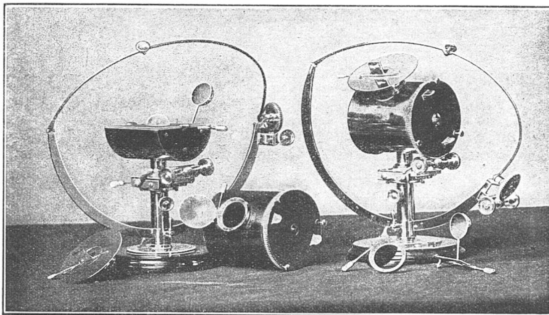
· PYRANOMÈTRE CONSTRUIT PAR LES SAVANTS AMÉRICAINS ABBOTT ET ALDRICH ·
