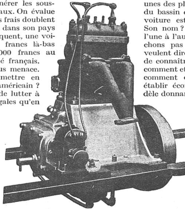
VUE EXTÉRIEURE DU MOTEUR A DEUX TEMPS, COTÉ DE L'ÉCHAPPEMENT
