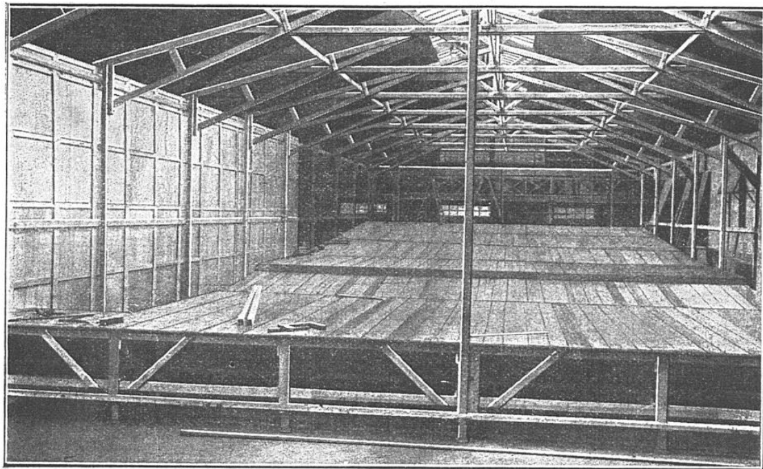
SALLE DE CINÉMA TRANSPORTABLE EN COURS DE MONTAGE
