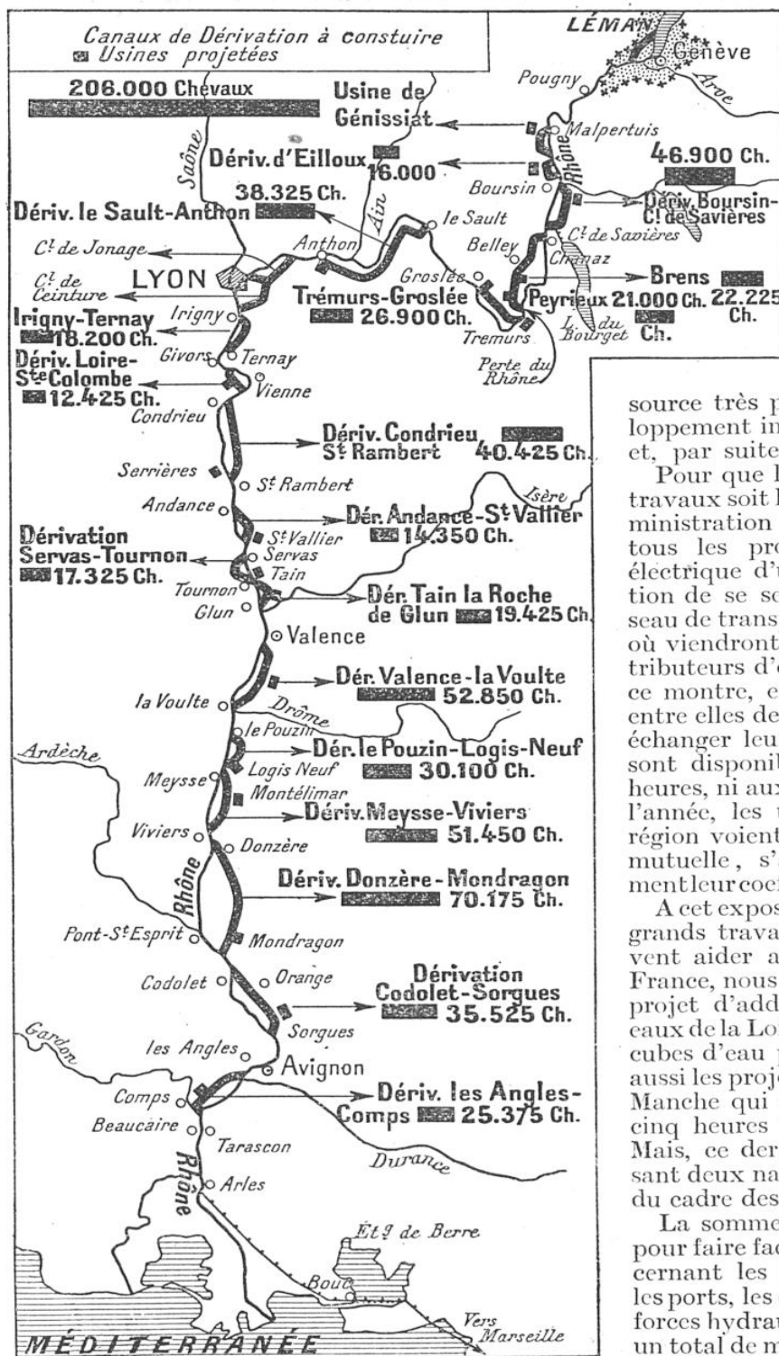
L'AMÉNAGEMENT DU COURS DU RHONE
