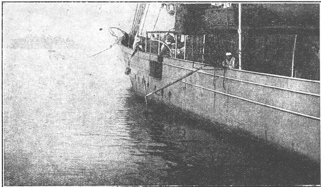
MISE A L'EAU, A BORD D'UN NAVIRE DE PATROUILLE, D'UN TUBE « C » AMÉRICAIN L'appareil se présente sous la forme d'un T renversé dont les deux petites branches sont munies chacune d'un diaphragme en caoutchouc. Le tube est emmanché sur le tuyau collecteur.
