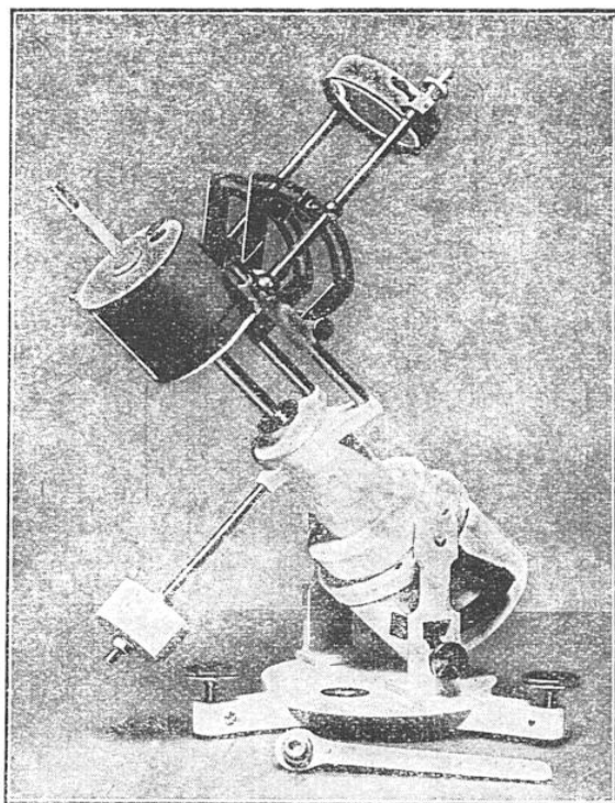
L'HÉLIOCHRONOGRAPHE DU DOCTEUR MAURER
