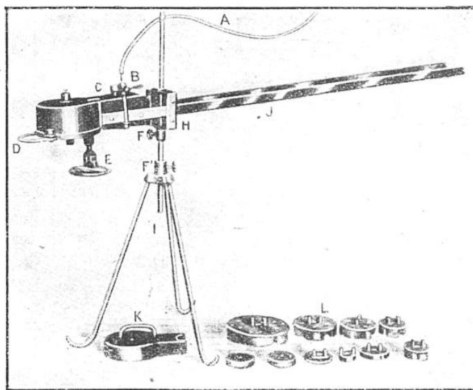
MACHINE GLAENZER SPÉCIALEMENT DESTINÉE A POLIR LE MARBRE ET LA PIERRE
