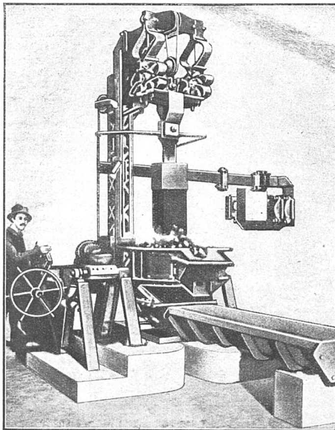
FOUR ÉLECTRIQUE DE 120 KILOWATTS
