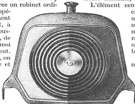
ADAPTATION DU NOUVEAU REFROIDISSEUR SUR UN RADIATEUR EN COUPE-VENT
