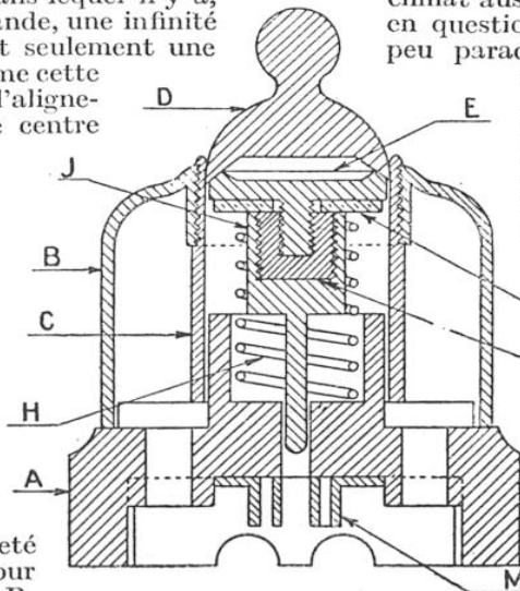
LORSQUE LE BOUTON D EST DROIT, ON SAIT QUE LE CIRCUIT EST COUPÉ
