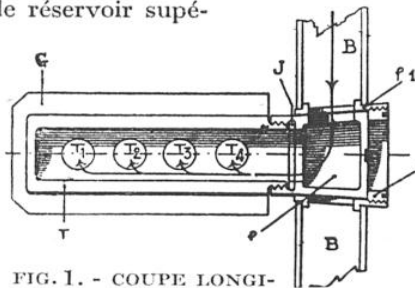
FIG. 1. - COUPE LONGITUDINALE D'UN DES COLLECTEURS
