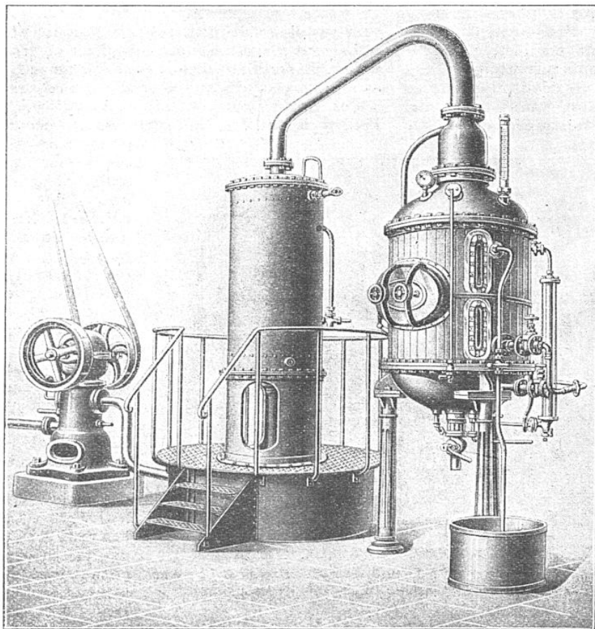
APPAREIL DESTINÉ A CONCENTRER LE LAIT DANS LE VIDE
