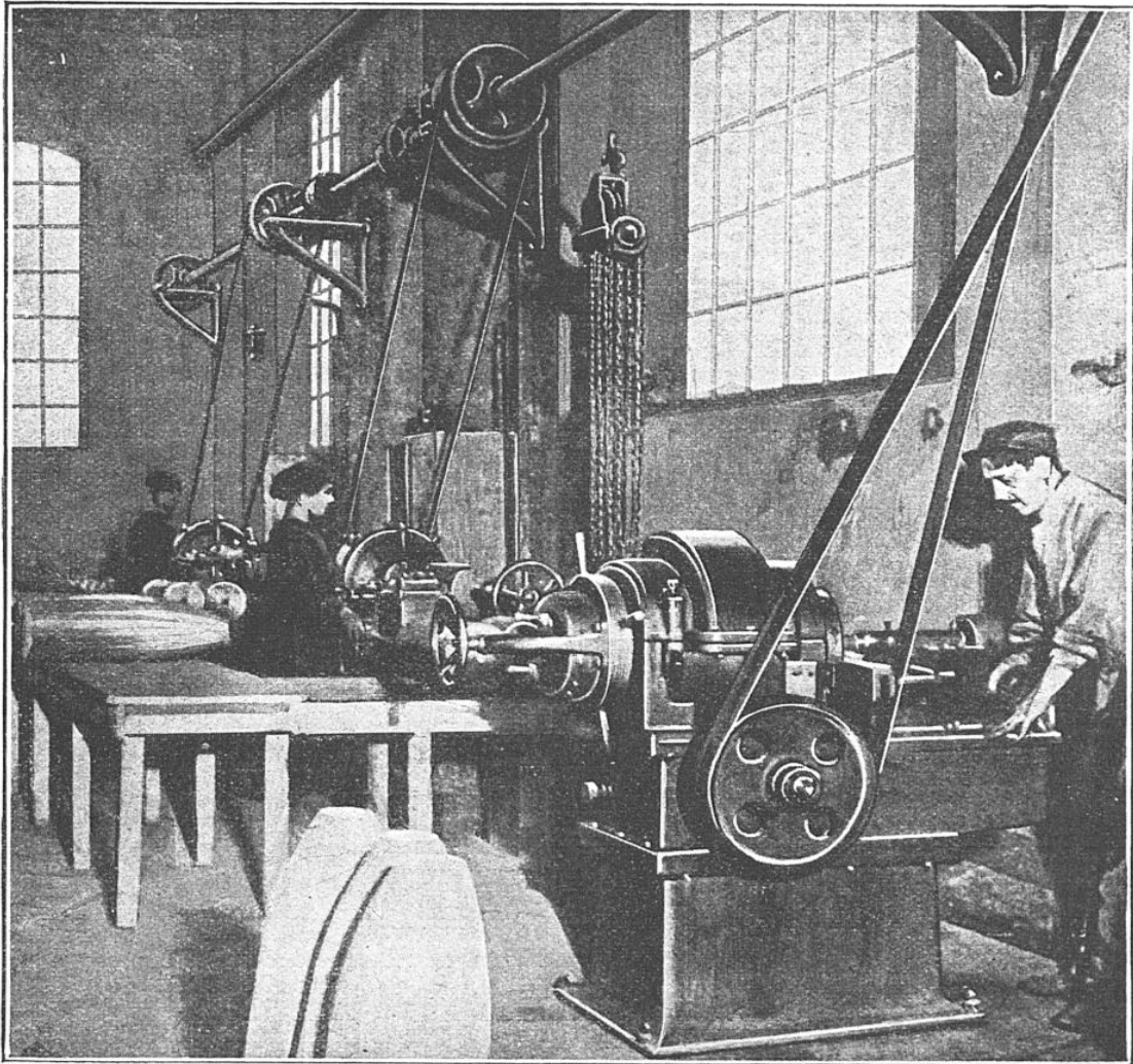
USINAGE DES OBUS DE 220 MILLIMÈTRES EN FONTE SYNTHÉTIQUE
