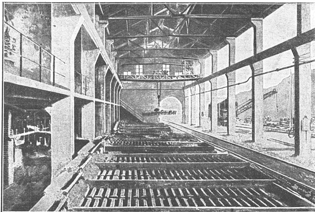
CHANTIERS DE COULÉE DE LA FONTE SYNTHÉTIQUE (FONDERIE DE NANTERRE)
