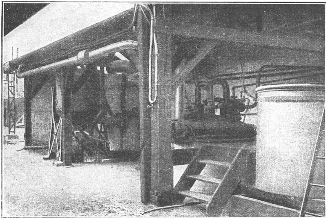
INSTALLATION POUR LA PRODUCTION RAPIDE, ET EN GRANDES QUANTITÉS, DU TOLUÈNE SULFOCHLORURÉ PAR MÉLANGES A CHAUD
