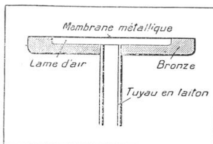
LE STÉTHOSCOPE DE M. BROCA
