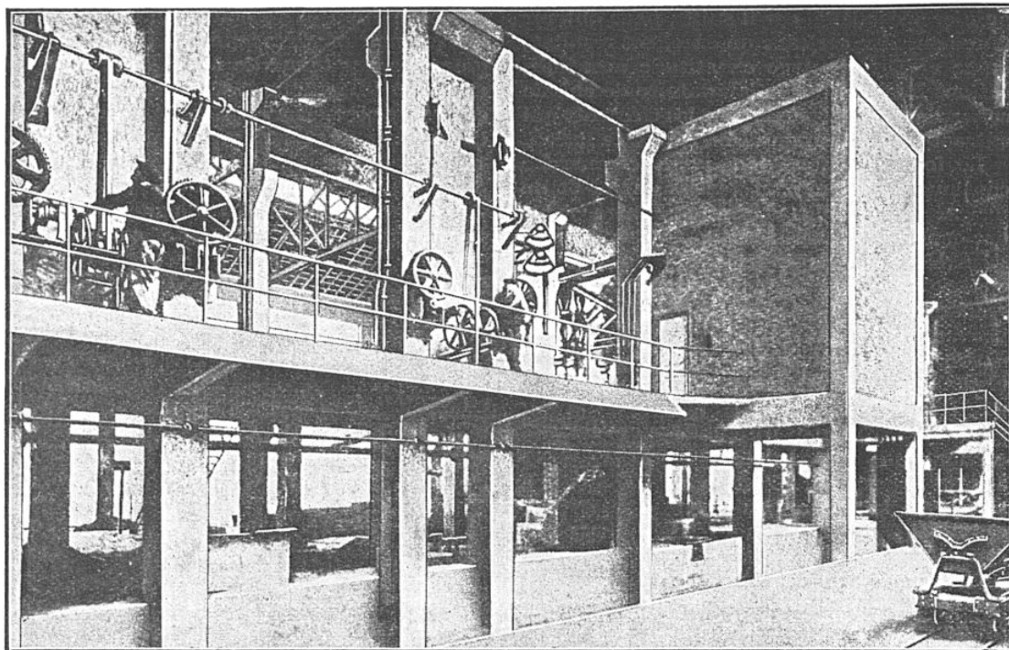
PLATE-FORME ET TREUILS POUR LE RÉGLAGE DES ÉLECTRODES (FONDERIE DE NANTERRE)
