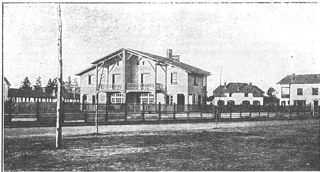
PHOTOGRAPHIE D'UN PAVILLON A UN ÉTAGE ET A QUATRE LOGEMENTS INDÉPENDANTS Les loggias avec balcons situées au rez-de-chaussée et au premier étage sont complètement séparées par un mur débordant. Chaque locataire est ainsi chez lui et ne peut être dérangé par ses voisins.
