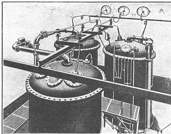
TRANSFORMATEURS DE 3.000 KILOWATTS, ISOLÉS A L'HUILE ET REFROIDIS PAR CIRCULATION D'EAU
