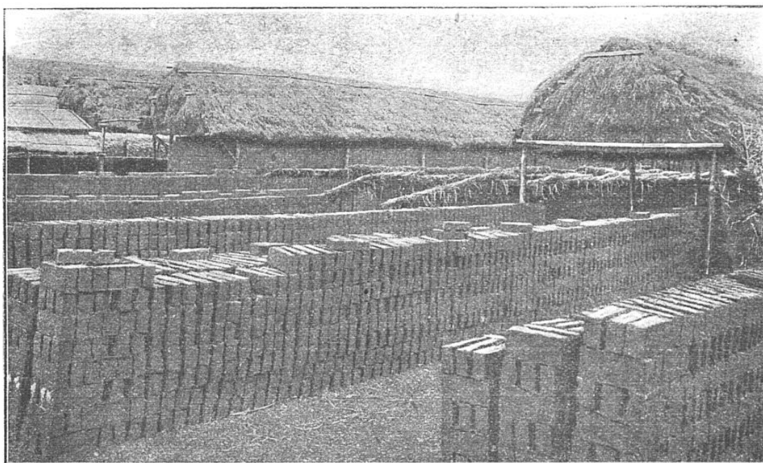
Le séchage des briquettes de terre de bruyère, disposées sur trois rangs superposés, se fait à l'air. Quand elles sont à peu près sèches, on les recouvre de roseaux.
