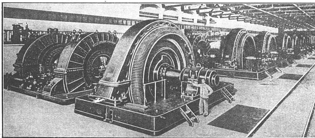
LA STATION GÉNÉRATRICE RENFERME 14 TURBINES JUMELÉES, QUI ENTRAÎNENT UN NOMBRE ÉGAL D'ALTERNATEURS TRIPHASÉS DE 12.000 VOLTS ET 25 PÉRIODES
