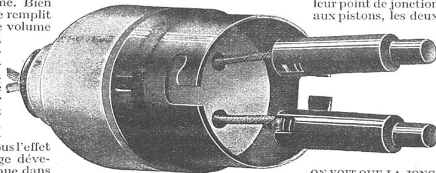
ON VOIT QUE LA JONCTION DES CONDUCTEURS AUX PISTONS NE NÉCESSITE AUCUNE VIS
