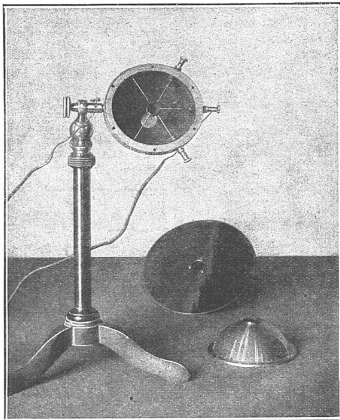
ACTINOMÈTRE FÉRY DÉMONTÉ
