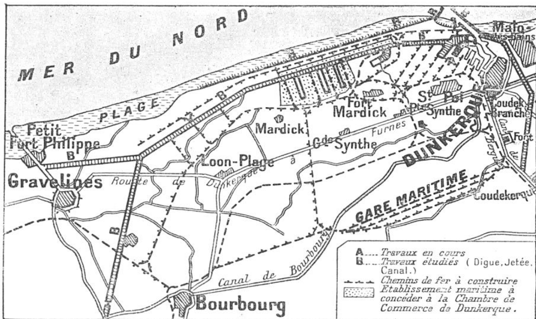
PLAN DU PORT DE DUNKERQUE AVEC L'INDICATION DES TRAVAUX PROJETÉS
