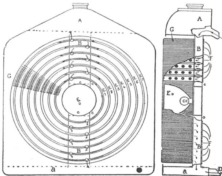
FIG. 3. - L'EAU CHAUDE PARVIENT DANS LE RÉSERVOIR A , PARCOURT LES ÉLÉMENTS E 1 E 2 E 3 , ETC., ARRIVE DANS LE RÉSERVOIR a , ET FAIT RETOUR AU MOTEUR
