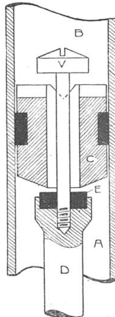
COUPE DU PISTON
