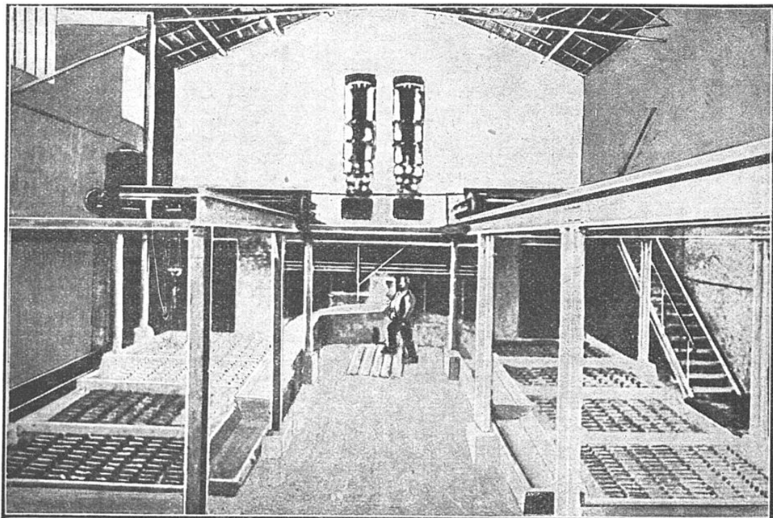
LE FOUR ÉLECTRIQUE ET LES CHANTIERS DE COULÉE DE L'USINE D'EYMOUTIERS
