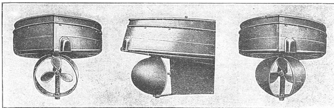
VUE ARRIÈRE ET VUE LATÉRALE DU GOUVERNAIL CORRESPONDANT A LA MARCHE EN AVANT A TOUTE VITESSE (POSITION DITE « OUVERTE »).
