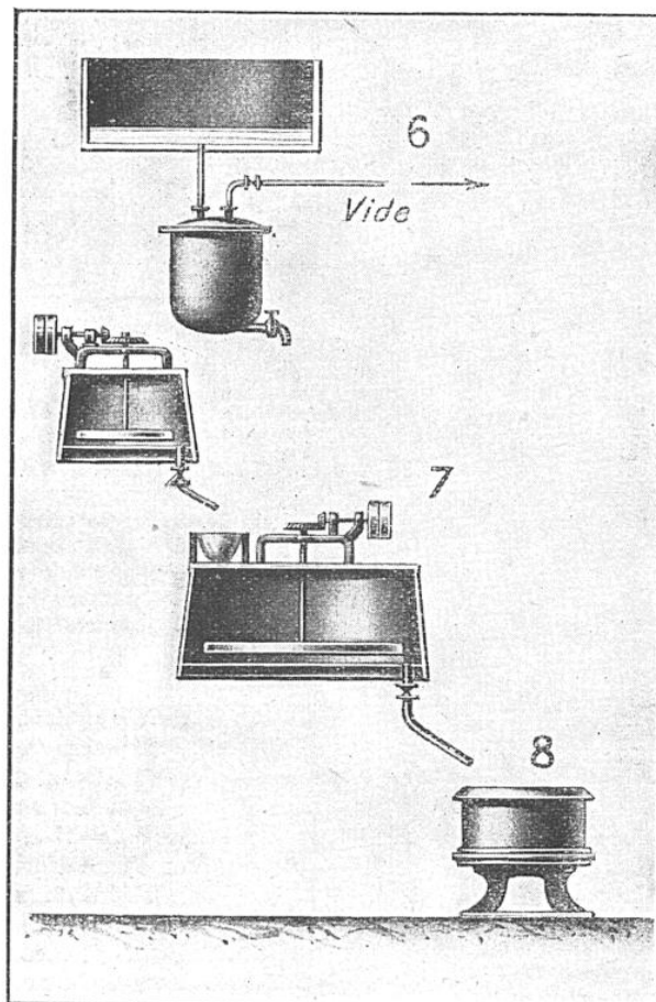
LES SIXIÈME, SEPTIÈME ET HUITIÈME OPÉRATIONS 6, isolement de l'amide brute ; 7 et 8, purification de l'amide.
