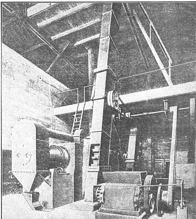
SÉCHEUR ROTATIF POUR LE COKE DE CARBURATION
