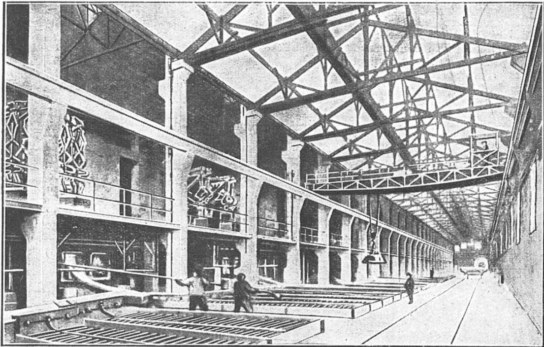
HALL DE FOURS ÉLECTRIQUES POUR FONTES SYNTHÉTIQUES (FONDERIE DE NANTERRE)
