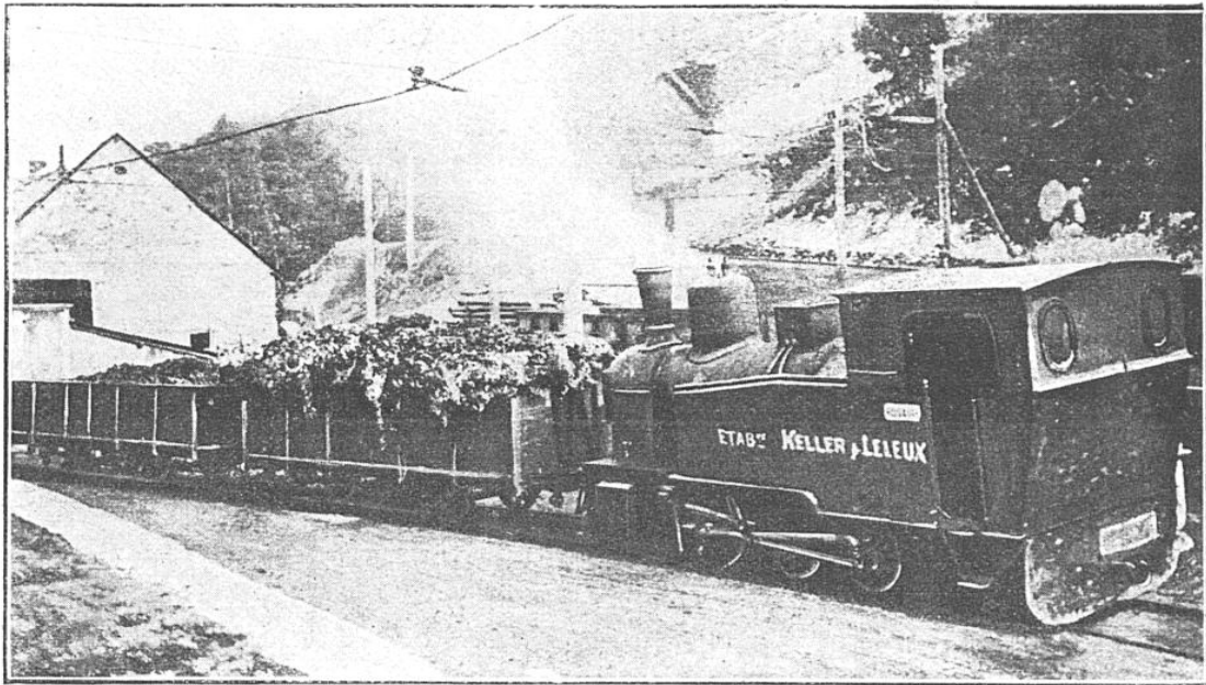
ARRIVÉE DE TOURNURES D'ACIER POUR LA FABRICATION DES FONTES SYNTHÉTIQUES PAR LE PROCÉDÉ KELLER, AUX USINES DE LIVET (ISÈRE)
