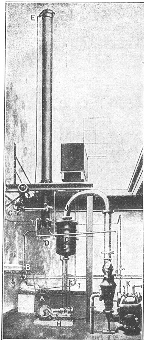
VUE GÉNÉRALE D'UN ÉVAPORATEUR KESTNER A FONCTIONNEMENT CONTINU
