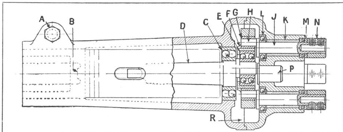
LES HUIT FORETS DE CES MANDRINS SONT ACTIONNÉS SIMULTANÉMENT PAR UN SYSTÈME DE MANIVELLES QUI ÉLIMINE COMPLÈTEMENT L'USAGE DES ENGRENAGES HABITUELS
