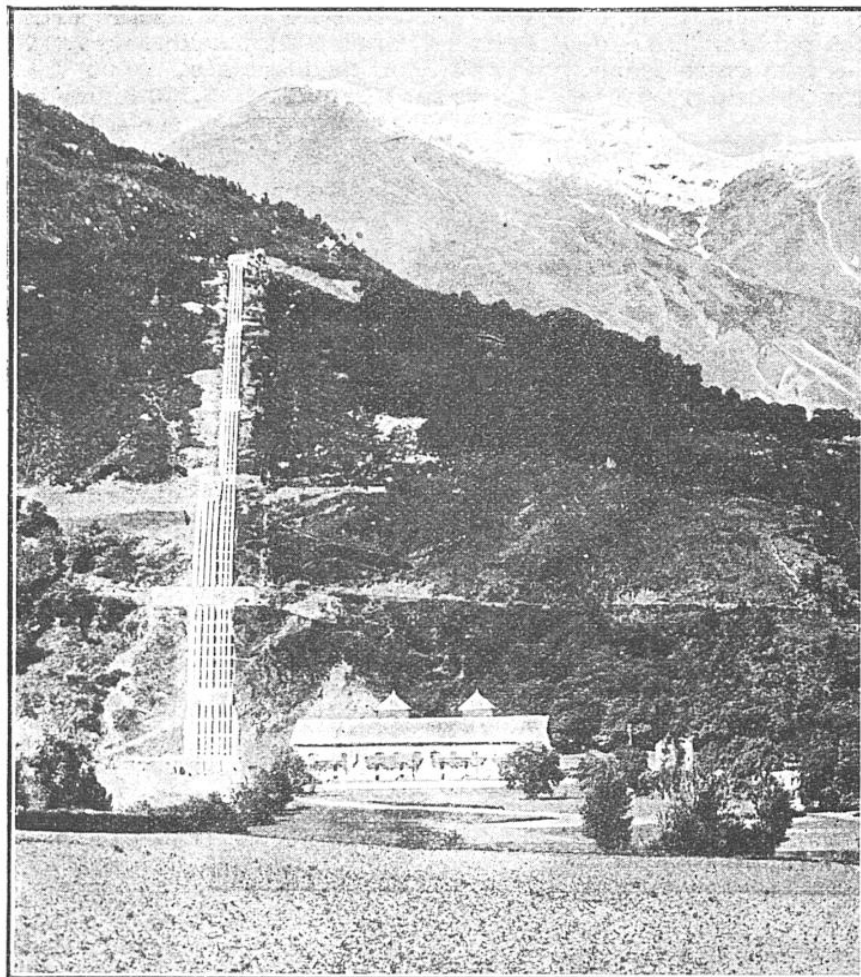
A L'USINE DE SOULOM, DE LA COMPAGNIE DES CHEMINS DE FER DU MIDI, LES EAUX PYRÉNÉENNES SONT AMENÉES PAR UNE REMARQUABLE CANALISATION QUE MONTRE NOTRE PHOTOGRAPHIE.
