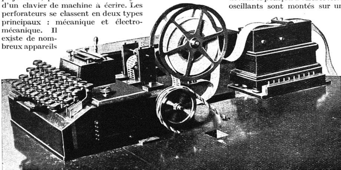
APPAREILS DE TRANSMISSION AUTOMATIQUE CARPENTIER ADAPTÉS AU BAUDOT
