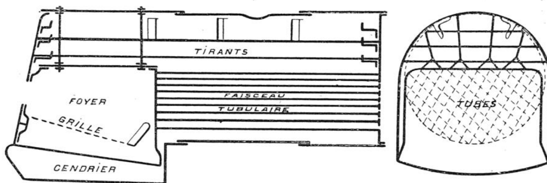
COUPE LONGITUDINALE ET COUPE TRANSVERSALE D'UNE CHAUDIÈRE LOCOMOTIVE
