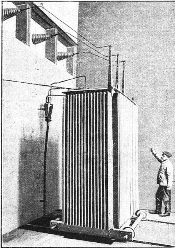
TRANSFORMATEUR TRIPHASÉ A BAIN D'HUILE, 5.500-65.000 VOLTS
