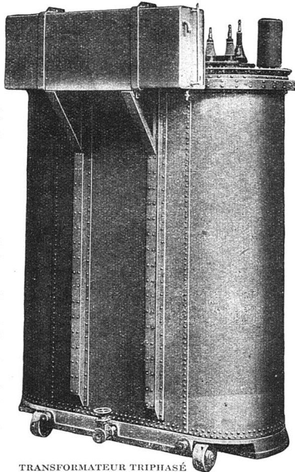
TRANSFORMATEUR TRIPHASÉ A REFROIDISSEMENT PAR CIRCULATION D'EAU Puissance : 6.000 kilowatts ; 52.500/10.000 volts. La cuve de cet appareil est hermétique et possède un réservoir d'expansion pour l'huile.
