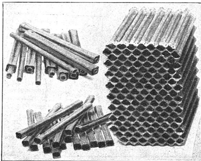
BLOC DE RADIATEURS EN TUBES LOBÉS
