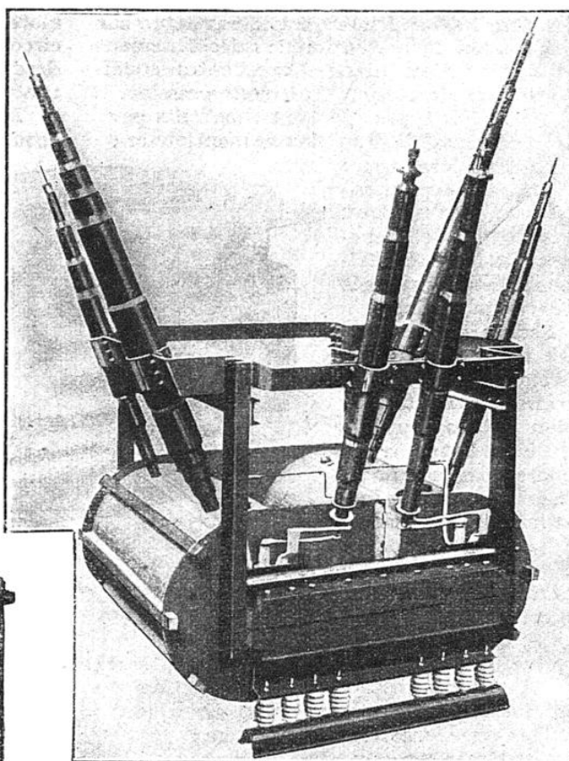
AUTRE TRANSFORMATEUR D'ESSAIS, MONOPHASÉ, DE 250.000 VOLTS, HORS DE SA CUVE
