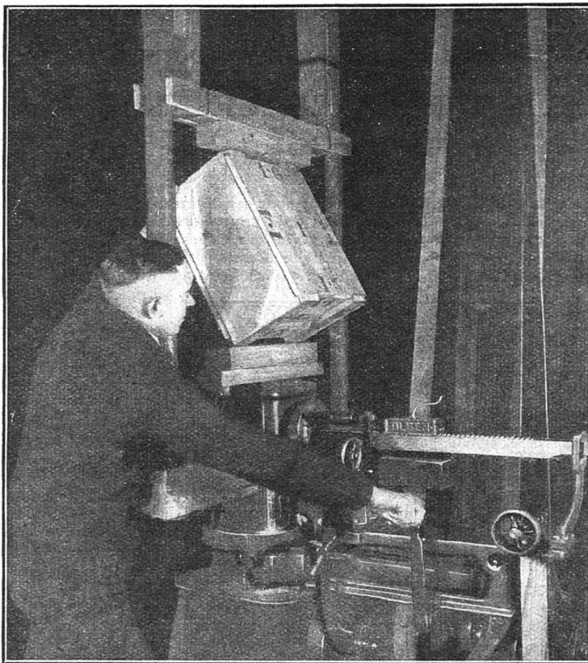
MACHINE A ESSAYER LA RÉSISTANCE DES CAISSES D'EMBALLAGE
