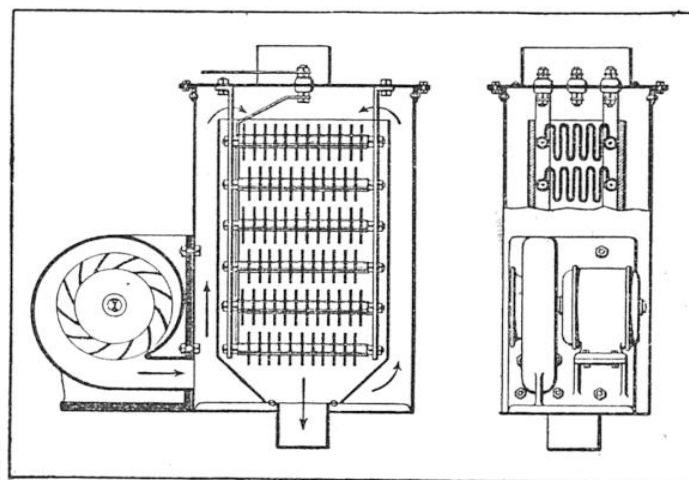
COUPE D'UN FOUR A AIR CHAUD DE 300 KILOWATTS, TRANSPORTABLE, POUR FONDERIE
