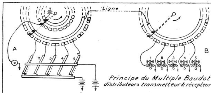
FIG. 2. — SCHÉMA DES CONNEXIONS AVEC DEUX POSTES
