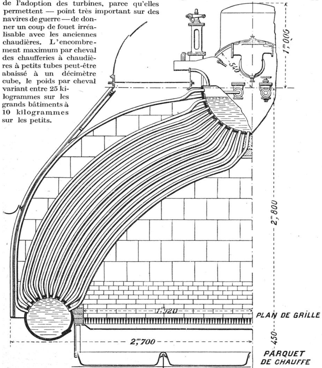
COUPE-ÉLEVATION DE LA CHAUDIÈRE AUGUSTIN NORMAND A RETOUR DE FLAMMES
