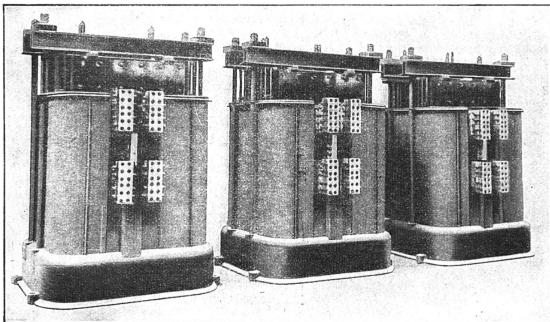
TROIS TRANSFORMATEURS MONOPHASÉS SE REFROIDISSANT PAR CIRCULATION D'AIR
