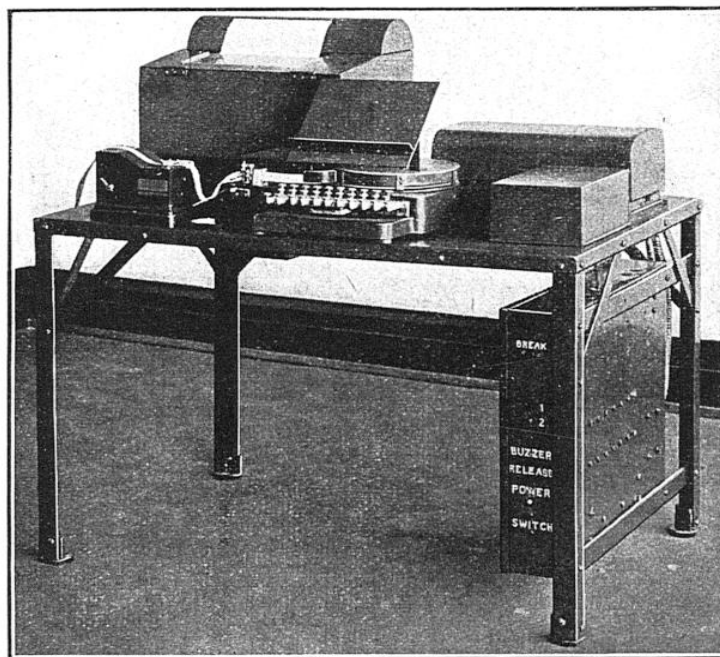
POSTE TRANSMETTEUR MORKRUM POUR LA DISTRIBUTION TÉLÉGRAPHIQUE DES NOUVELLES DE PRESSE
