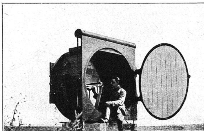
LES PROJECTEURS DE CETTE DIMENSION (1 M. 50) PERMETTENT DES PORTÉES TÉLÉGRAPHIQUES DE 25 KILOMÈTRES
