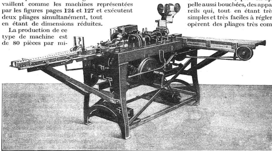
MACHINE SPÉCIALE POUR L'EMPAQUETAGE DES CUBES DE BOUILLON
