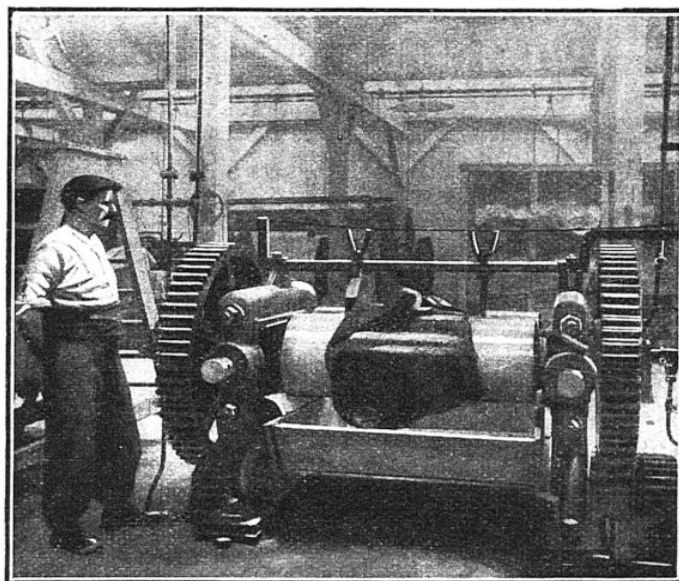
LAMINOIR A CYLINDRES LISSES SERVANT A AGGLOMÉRER LES FRAGMENTS DE CAOUTCHOUC
