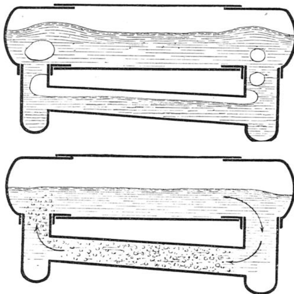
DANS LA PREMIÈRE FIGURE, LA VAPEUR CIRCULE MAL ET PAR A-COUPS ; DANS LA SECONDE, LA CIRCULATION EST ACTIVE ET CONTINUE
