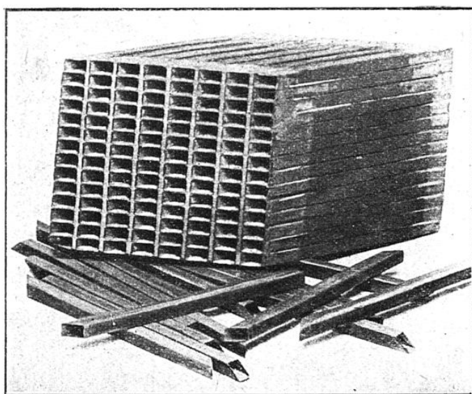
LE PREMIER TYPE DE RADIATEUR « NID D'ABEILLES » Il se compose d'une série de tubes carrés soudés entre eux par leurs extrémités et séparés par une tige de cuivre dont l'épaisseur sert à ménager l'espace nécessaire au passage de l'eau.
