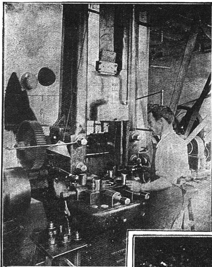
MOUTON POUR LA FRAPPE DES BOÎTES DE MONTRES
