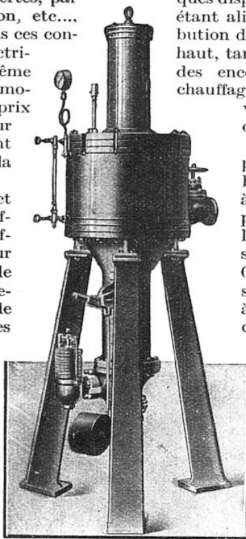
NOUVEAU FOUR ÉLECTRIQUE DE L'INGÉNIEUR REVEL
