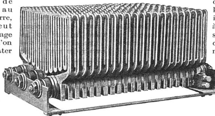
ÉLÉMENTS DE CHAUFFAGE ÉLECTRIQUE COMPOSÉS DE SÉRIES DE RÉSTANCES EN FONTE SPÉCIALE, POUR INSTALLATIONS INDUSTRIELLES
