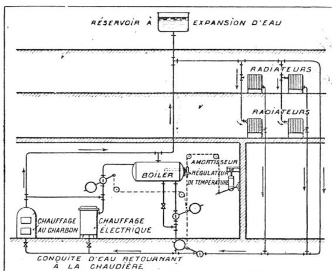
CHAUFFAGE CENTRAL ÉLECTRIQUE AVEC ACCUMULATION DE CHALEUR, DIT A DISTRIBUTION RETARDÉE Système combiné avec une chaudière à charbon.
