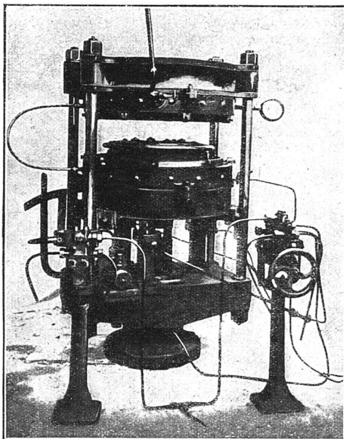
PRESSE SPÉCIALE POUR LA FABRICATION DES PNEUMATIQUES DE BICYCLETTES
