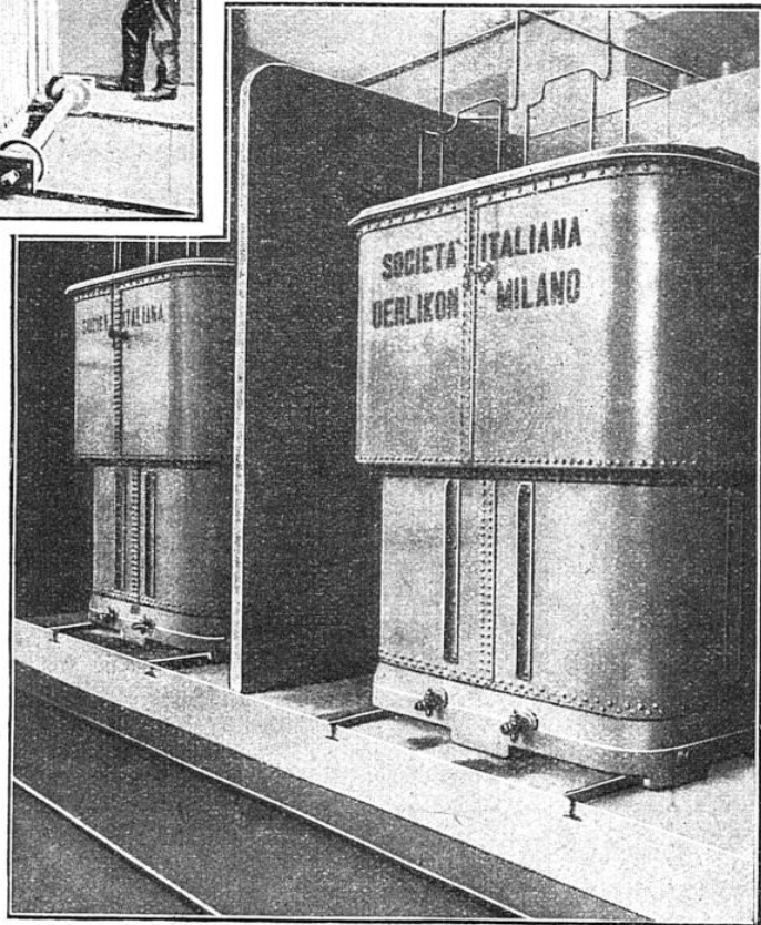
TRANSFORMATEURS TRIPHASÉS DANS LEUR CUVE A HUILE (Société italienne pour l'utilisation des forces du Veneto (Vénétie)).
