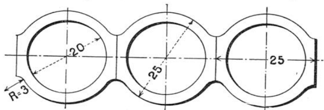
TUBES SPÉCIAUX POUR LES RANGÉES JOINTIVES DANS LES CHAUDIÈRES SYSTÈME NORMAND
