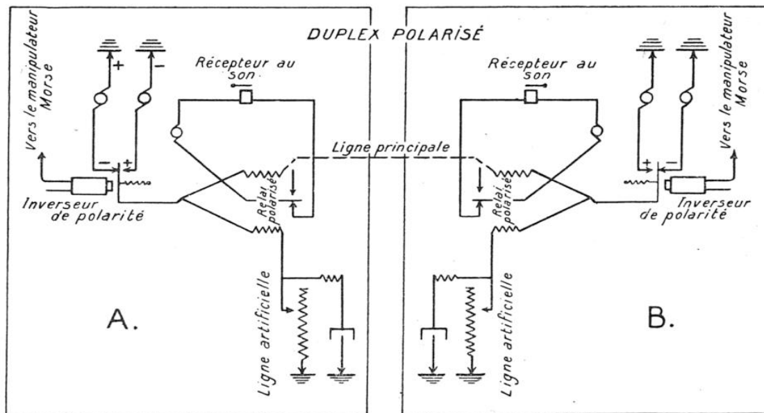
FIG. 4. — L'EXPLOITATION D'UNE LIGNE EN DUPLEX PERMET, AU MOYEN D'UN SEUL FIL, DE TRANSMETTRE ET DE RECEVOIR SIMULTANÉMENT UN MESSAGE
