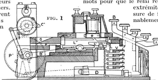
FIG. 1. COUPE DU PERFORATEUR MÉCANIQUE CARPENTIER
