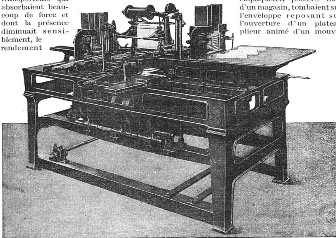
TYPE DE MACHINE A ENVELOPPER LES TABLETTES DE CHOCOLAT
