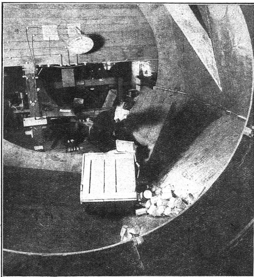
COMPLÈTEMENT DÉMOLIE AU COURS D'UN ESSAI, CETTE CAISSE LAISSE ÉCHAPPER SON CONTENU DE BOÎTES DE CONSERVES
