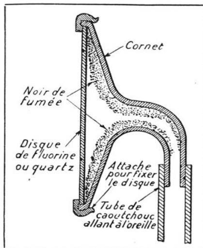
CETTE CAPSULE TRANSFORME EN ONDES SONORES LES ONDES INFRA-ROUGES QUI TOMBENT SUR ELLE
