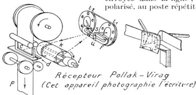
FIG. 7. — LES COURANTS PARVENANT AU POSTE RÉCEPTEUR METTENT EN MOUVEMENT UN MIROIR QUI, EN RÉFLÉCHISSANT UN RAYON LUMINEUX, TRACE L'ÉCRITURE SUR UNE BANDE DE PAPIER SENSIBLE
