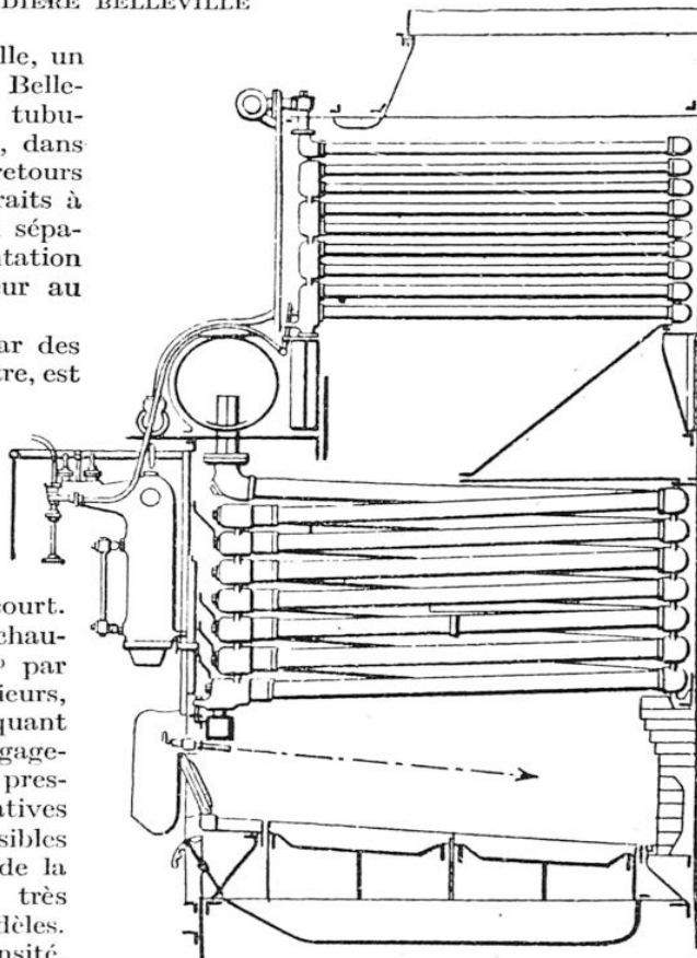
CHAUDIÈRE BELLEVILLE DU TYPE MODERNE
