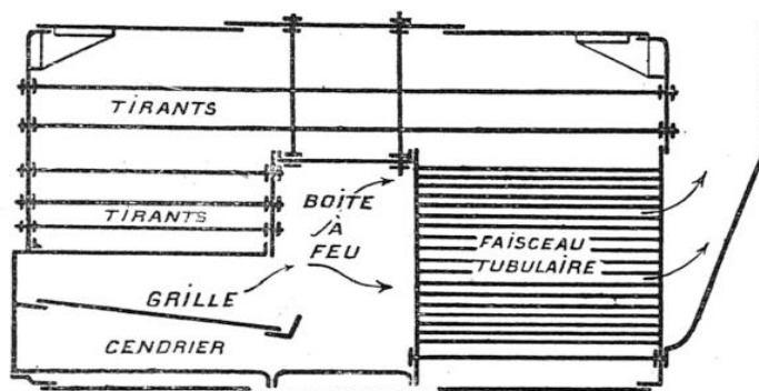
COUPE D'UNE CHAUDIÈRE DITE DE L'AMIRAUTÉ
