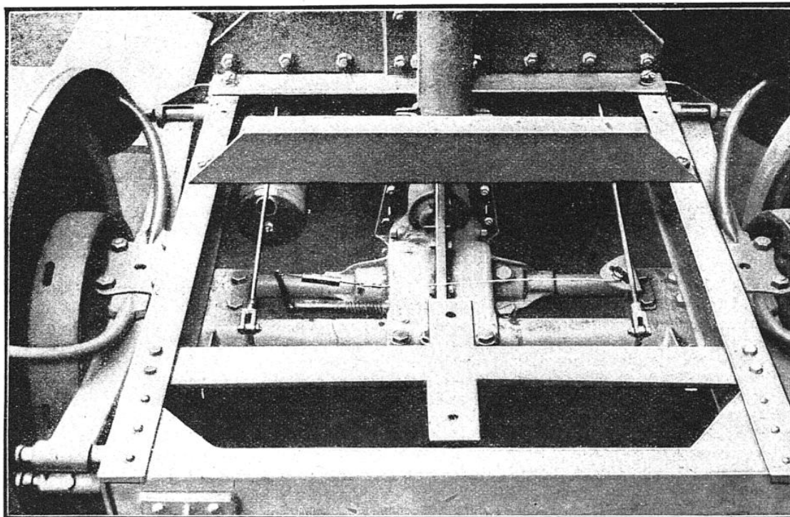
VUE DE L'ARRIÈRE DU TRACTEUR ET DE SON ESSIEU MOTEUR
