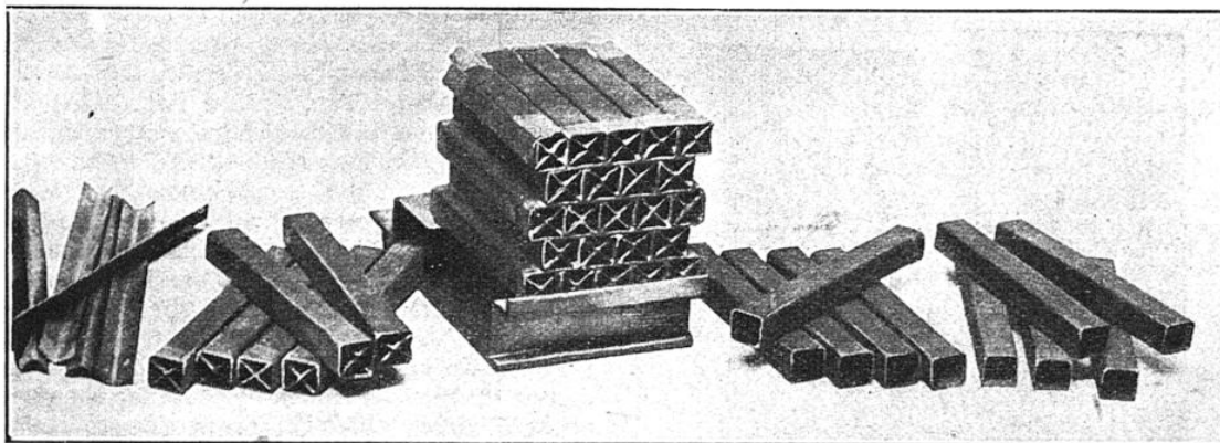
« NID D'ABEILLES » AVEC ADDITION DE FEUILLES DE CUIVRE A L'INTÉRIEUR DES TUBES
