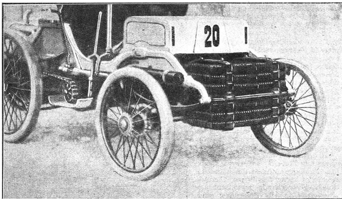
TYPE DE RADIATEUR TEL QU'ON LE FAISAIT IL Y A UNE VINGTAINE D'ANNÉES Un serpentin garni d'ailettes rapportées sur le tube était placé à l'avant de la voiture, de façon à refroidir activement l'eau de circulation du moteur.
