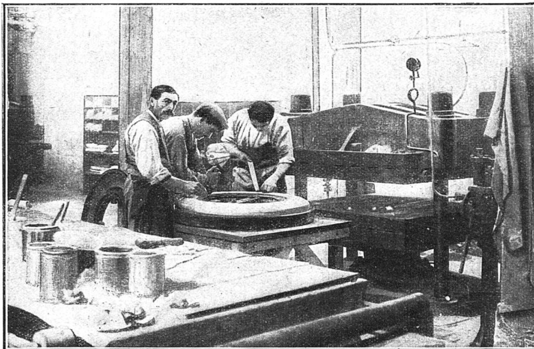
L'ESTAMPAGE A FROID D'UNE ENVELOPPE DE PNEUMATIQUE
