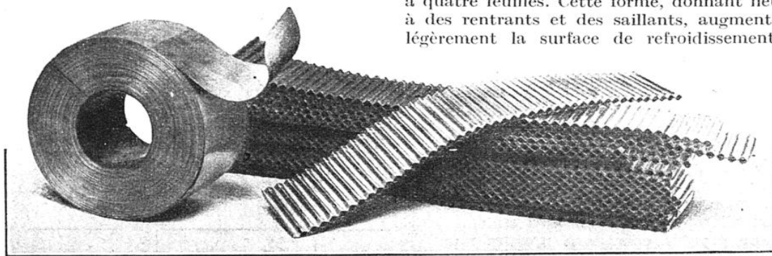
MODE DE FABRICATION D'UN RADIATEUR SYSTÈME MOREUX
