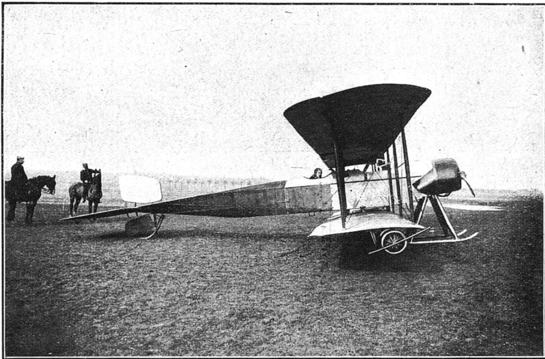
L'INCIDENCE VARIABLE A ÉTÉ RÉALISÉE, DÈS 1912, SUR L'AÉROPLANE SCHMITT Quand l'appareil est en plein vol, on réduit au minimum l'incidence de la cellule, de façon à obtenir le maximum de vitesse dans un temps relativement très court.
