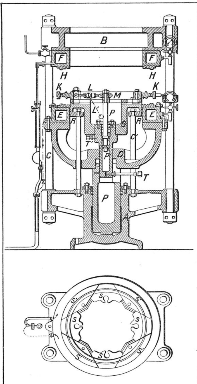
VUE EN COUPE ET EN PLAN DE LA PRESSE A VÉLO
