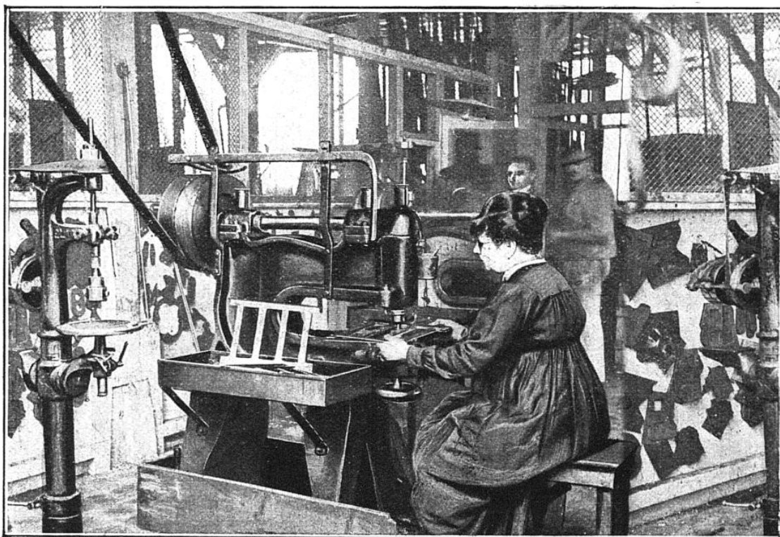
VUE GÉNÉRALE DE LA MACHINE MOREUX POUR LE DÉCOUPAGE DES TÔLES
