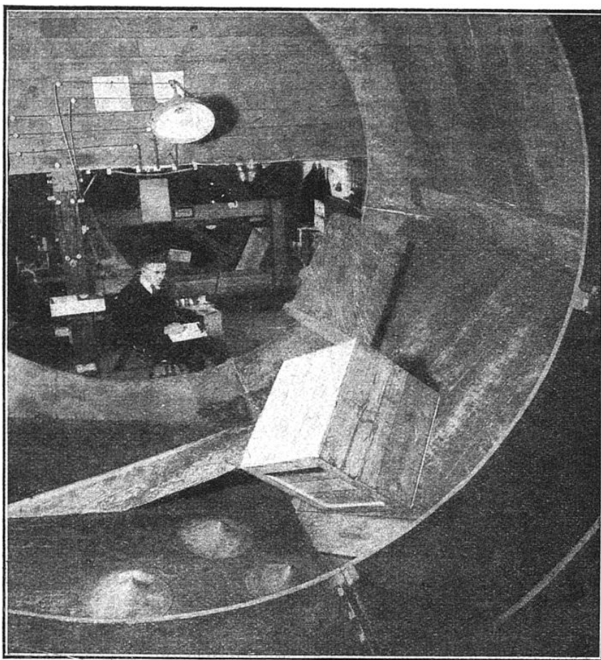
TAMBOUR TOURNANT DU « FOREST PRODUCTS LABORATORY »
