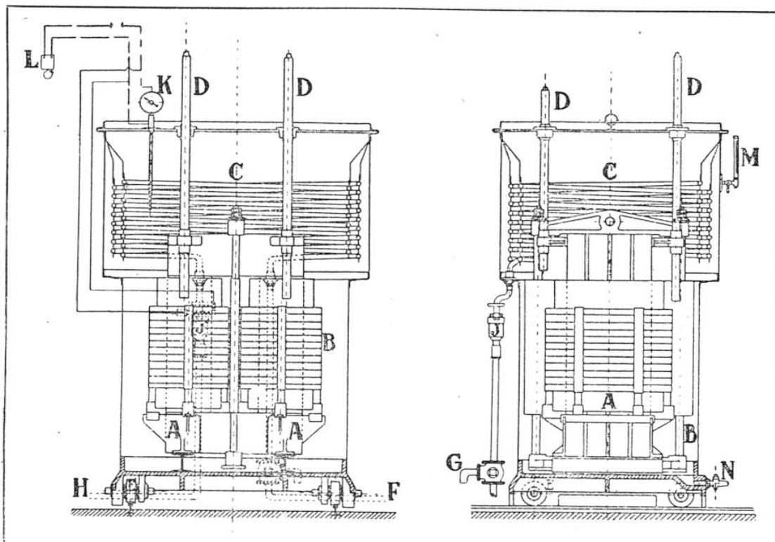
COUPE LONGITUDINALE ET COUPE TRANSVERSALE D'UN TRANSFORMATEUR MONOPHASÉ A BAIN D'HUILE, AVEC REFROIDISSEMENT PAR CIRCULATION D'EAU
