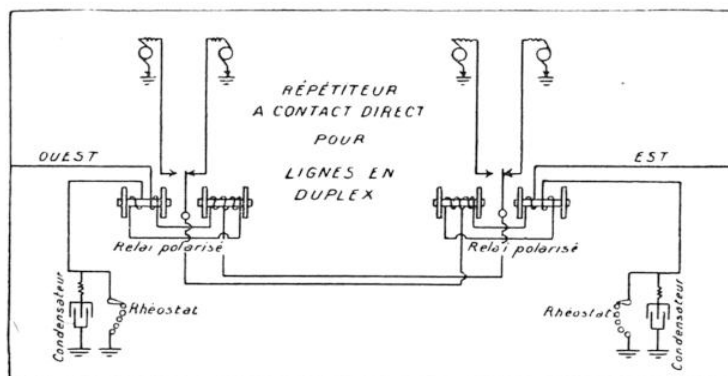
FIG. 6. — LES RÉPÉTITEURS SERVENT À RENFORCER L'INTENSITÉ DES SIGNAUX SUR LES LIGNES DE GRANDE LONGUEUR
