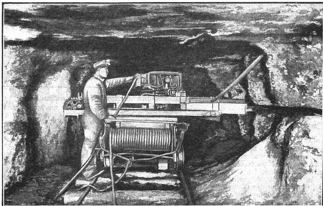
HAVEUSE MÉCANIQUE MONTÉE SUR CHARIOT POUR L'ABATAGE DU CHARBON
