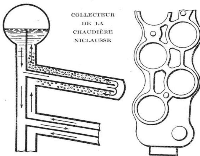
Ce collecteur est divisé en deux parties ; de la partie gauche l'eau d'alimentation se rend dans le tube directeur et l'eau et la vapeur produite par réchauffement du tube vaporisateur montent dans la partie droite du collecteur.
