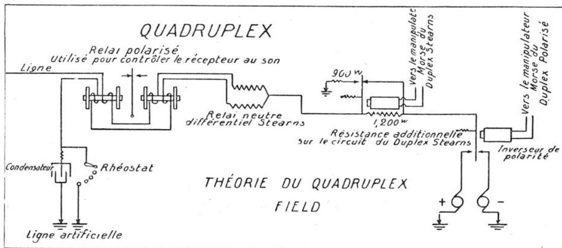
FIG. 5. — LE QUADRUPLIX PERMET DE TRANSMETTRE, TOUJOURS PAR LE MÊME FIL ET AU MÊME INSTANT, DEUX SIGNAUX DANS CHAQUE DIRECTION
