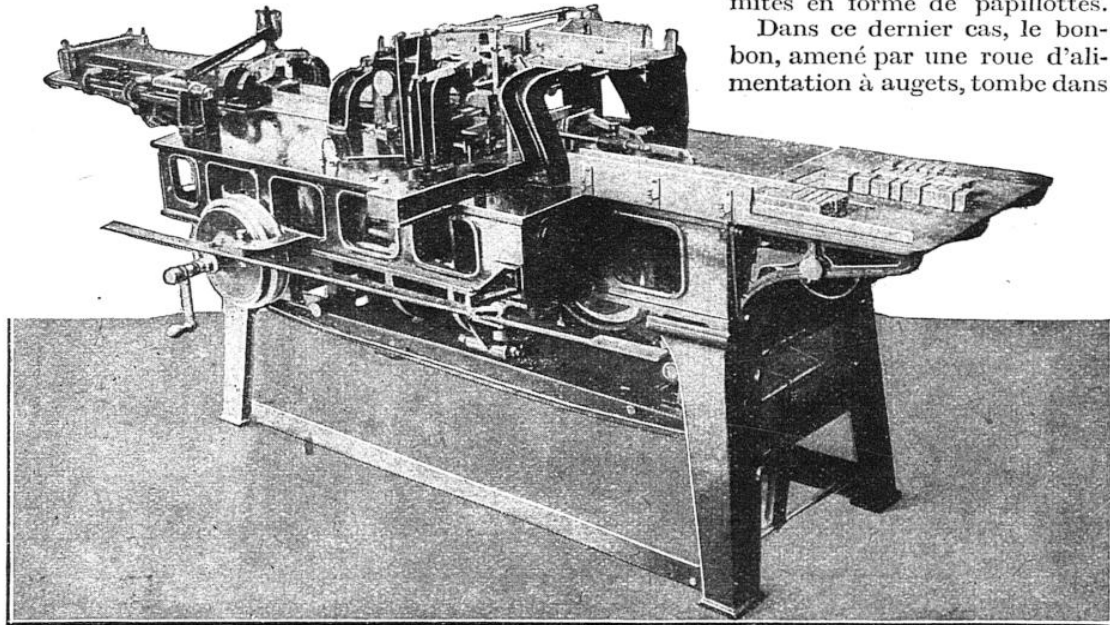
MACHINE SERVANT A FAIRE LES PAQUETS DE DIX BISCUITS
