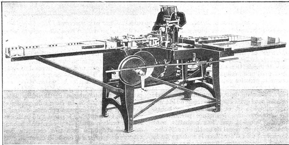
APPAREIL SERVANT A EMBALLER LES BLOCS DE SAVON EN BOITES PLIANTES
