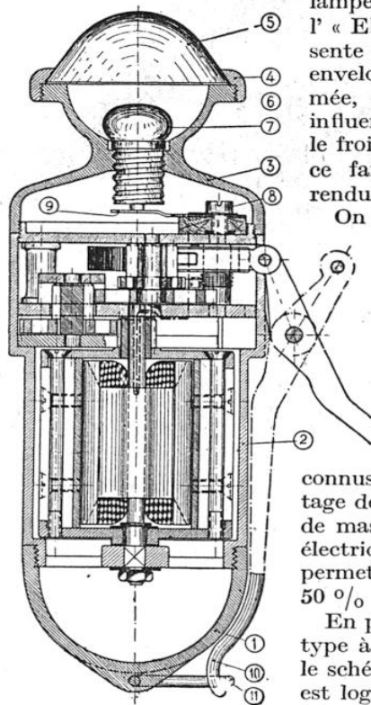
COUPE LONGITUDINALE DE LA LAMPE « ÉLECTRO-AUTOMATE »
