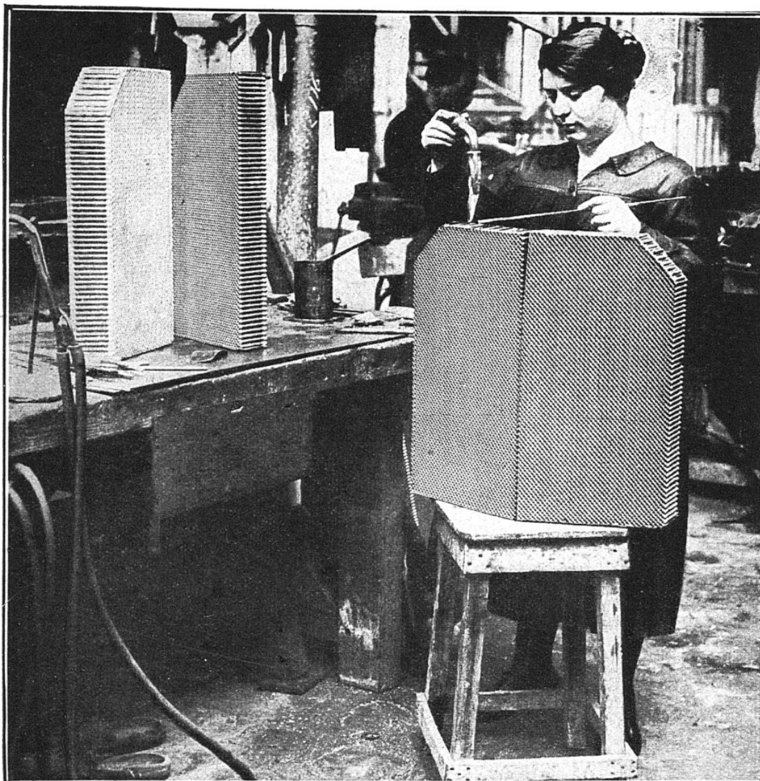
FABRICATION D'UN BLOC DE RADIATEUR A BANDES
