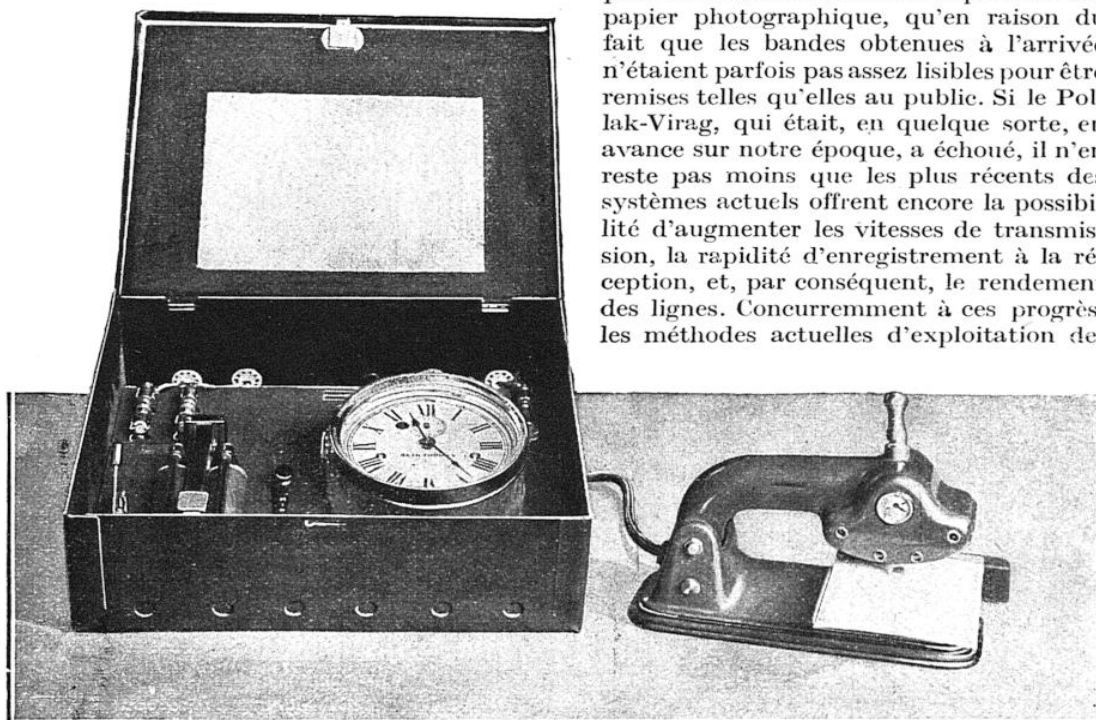
L'HEURE AUSSI BIEN QUE LA DATE SONT, AUX ÉTATS-UNIS, TIMBRÉES SUR LES TÉLÉGRAMMES Le dateur-horaire est contrôlé électriquement, ainsi que sa montre-témoin, par une horloge mère qui se remonte automatiquement et peut commander, au moyen de relais, autant de timbres qu'on veut.
