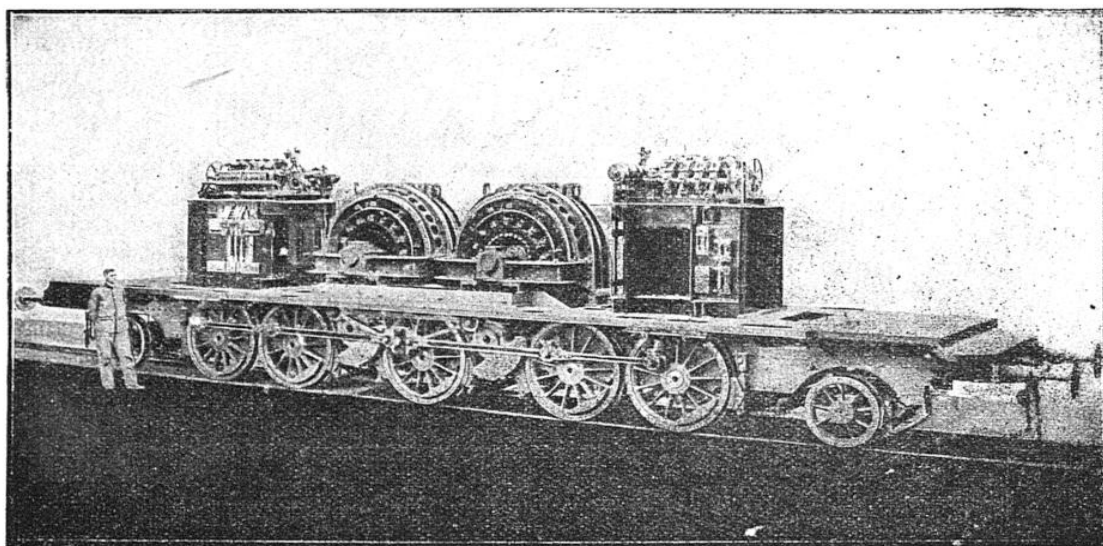
CHASSIS DE LOCOMOTIVE ÉLECTRIQUE A SEPT PAIRES DE ROUES, AVEC DEUX MOTEURS AU CENTRE ET UN TRANSFORMATEUR A CHAQUE EXTRÉMITÉ
