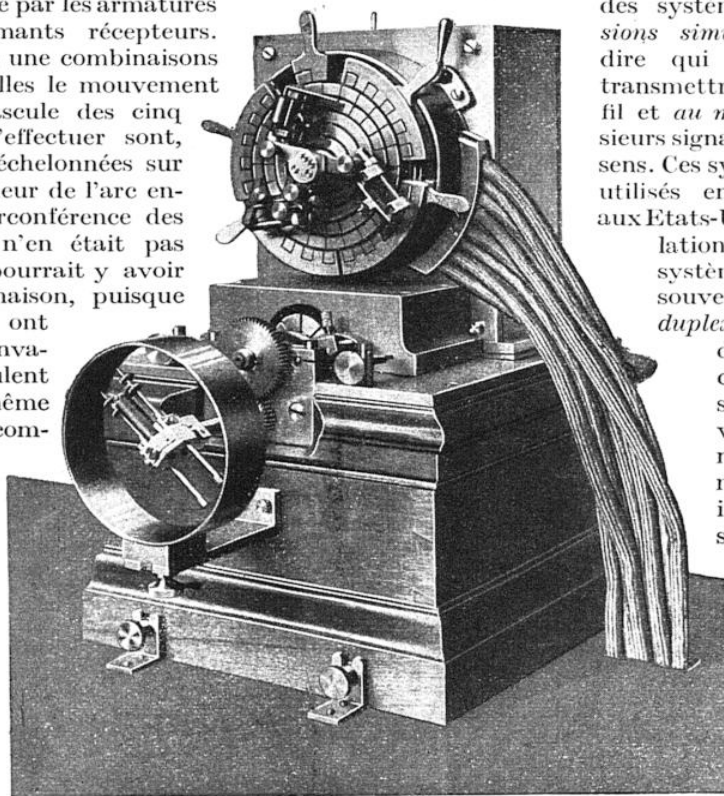
DISTRIBUTEUR CARPENTIER POUR TRANSMISSION OU RÉCEPTION SUR LIGNE EXPLOITÉE EN QUADRUPLE BAUDOT
