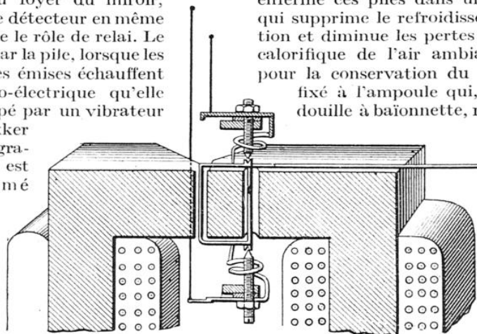
GALVANOMÈTRE A GRANDE SENSIBILITÉ POUR LA DÉTECTION (RECHERCHE) DES NAVIRES ET DES ICEBERGS
