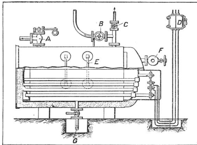
CHAUDIÈRE ÉLECTRIQUE GARNIE DE CALORIFÈGE POUR PRODUCTION DE VAPEUR A UTILISATION RETARDÉE
