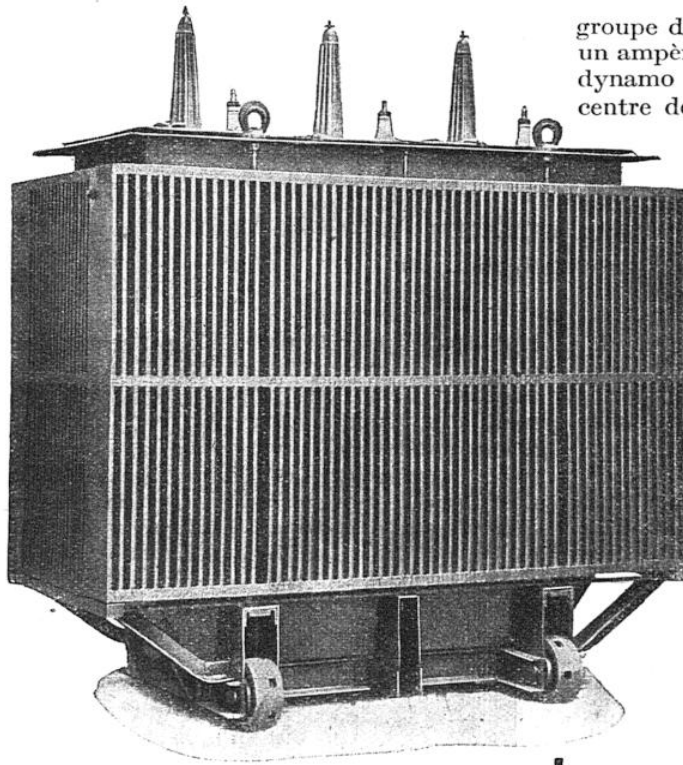
TRANSFORMATEUR TRIPHASÉ A BAIN D'HUILE ET REFROIDISSE- MENT NATUREL 3.300-40.000 volts ; 50 périodes.
