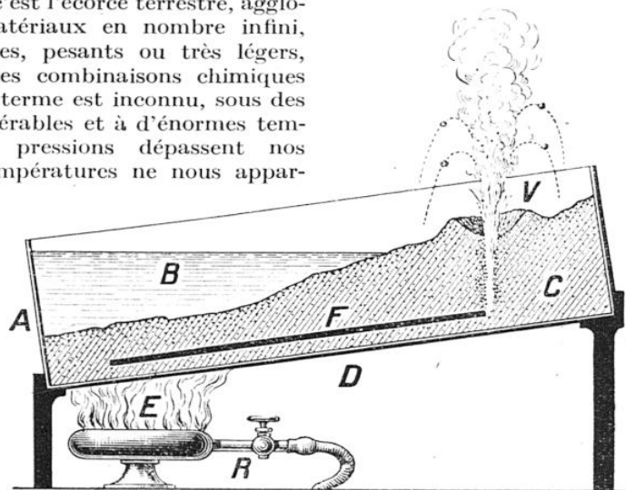
LE BASSIN EXPÉRIMENTAL DE M. BELOT (COUPE)
