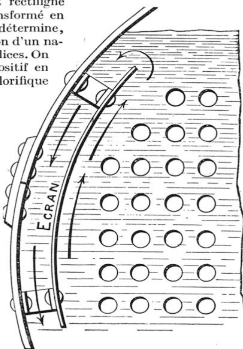
DISPOSITIF IMAGINÉ PAR M. AUGUSTIN NORMAND POUR AMENER UNE CIRCULATION LOGIQUE DE L'EAU DANS LES CHAUDIÈRES A VAPEUR
