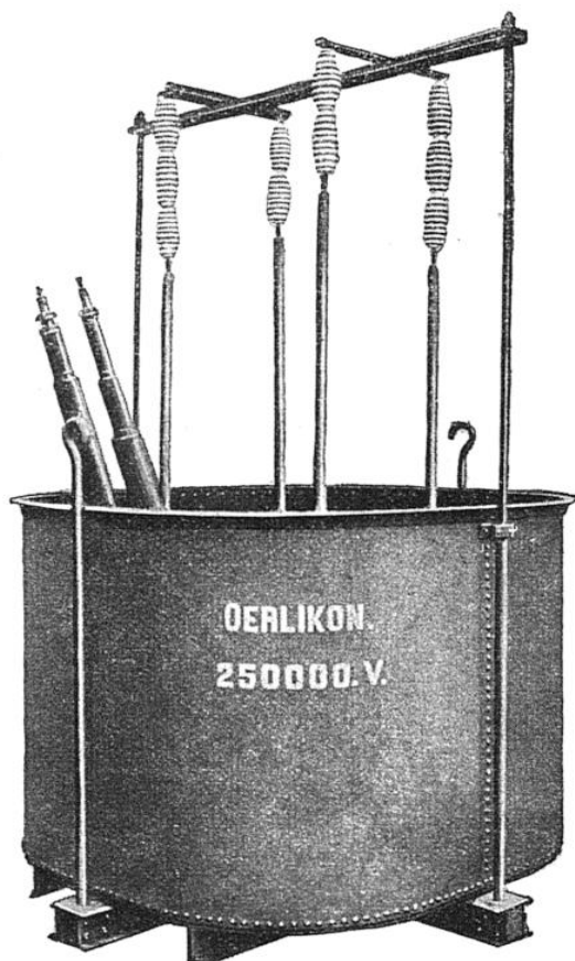
TRANSFORMATEUR D'ESSAIS, MONOPHASÉ, DE 250.000 VOLTS, PLACÉ DANS SA CUVE
