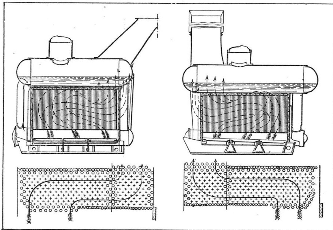
DEUX TYPES DE CHAUDIÈRES CONSTRUITES PAR M. AUGUSTIN NORMAND
