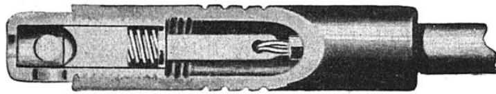
DISPOSITIF INTÉRIEUR DE LA FICHE DE CONTACT
