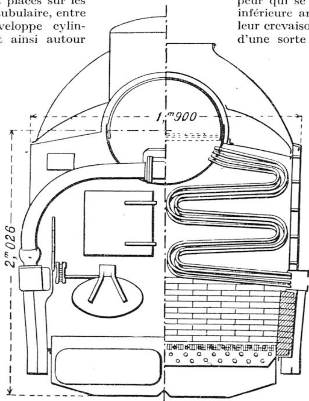
CHAUDIÈRE PRIMITIVE DU « TEMPLE »
