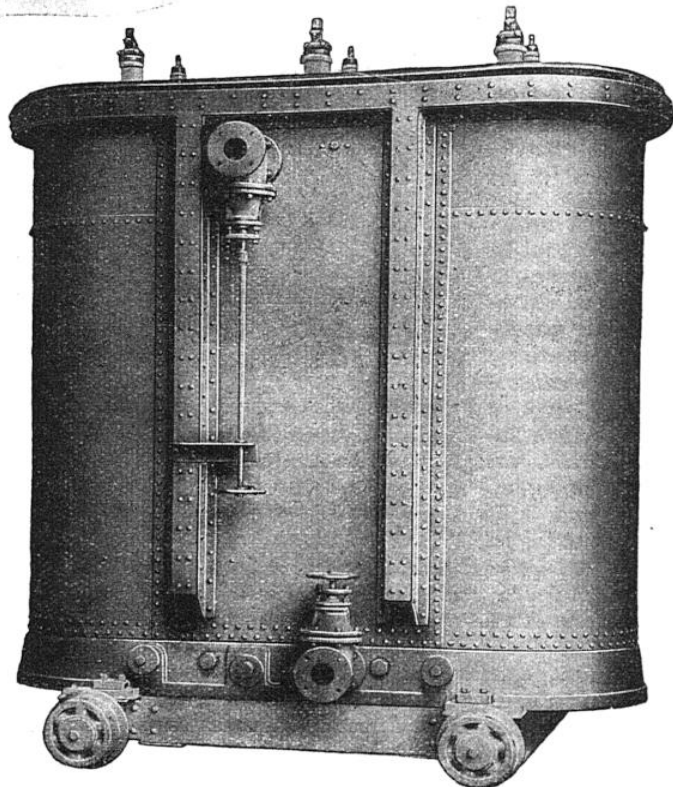
TRANSFORMATEUR TRIPHASÉ DANS SA CUVE A HUILE, AVEC REFROIDISSEMENT PAR EAU
