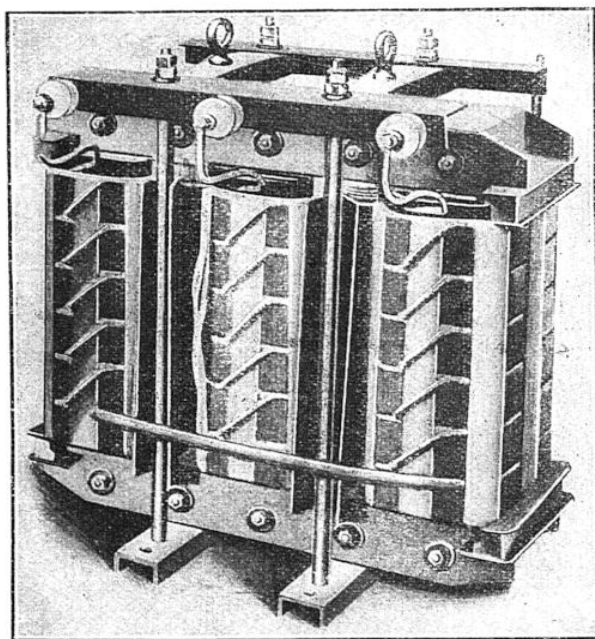
TRANSFORMATEUR TRIPHASÉ, AVEC REFROIDISSEMENT PAR CIRCULATION D'EAU
