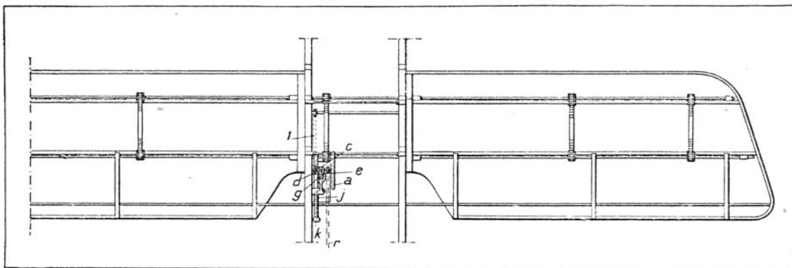
STRUCTURE DE L'AILE INFÉRIEURE DE L'AÉROPLANE DHUMBERT
