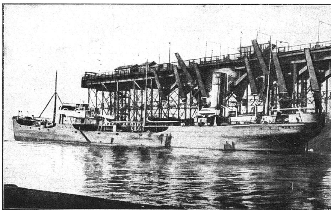
POSTE DE CHARGEMENT MÉCANIQUE DE CHARBON DANS UN PORT AMÉRICAIN
