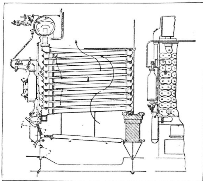
CONCEPTION PRIMITIVE DE LA CHAUDIÈRE BELLEVILLE
