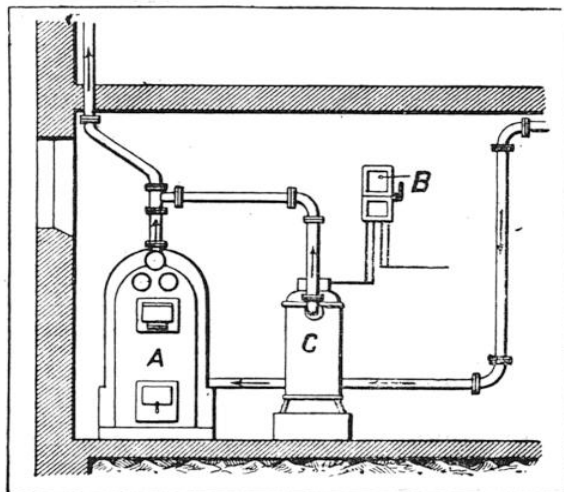
CHAUFFAGE CENTRAL A EAU CHAUDE, AVEC CHAUDIÈRE ÉLECTRIQUE DE SECOURS
