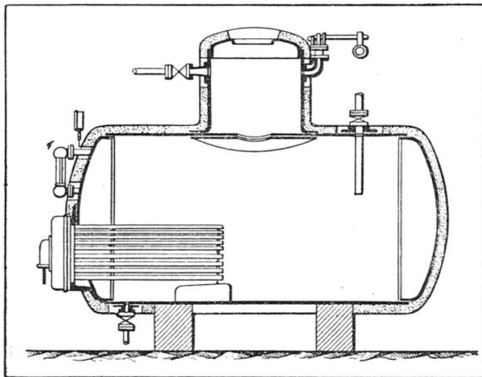
COUPE D'UNE CHAUDIÈRE ÉLECTRIQUE DE 500 KILOWATTS POUR LA PRODUCTION DE VAPEUR
