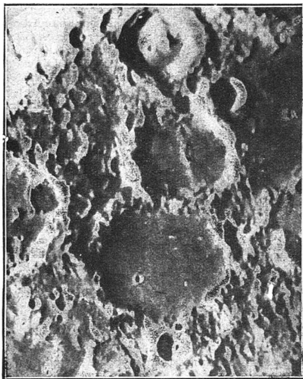
LE CRATÈRE LUNAIRE « PTOLÉMÉE »
