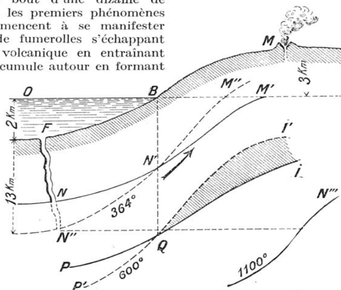
FIGURE SCHÉMATIQUE EXPLIQUANT LE RELÈVEMENT DES SURFACES ISOTHERMES SOUS LES CONTINENTS.
