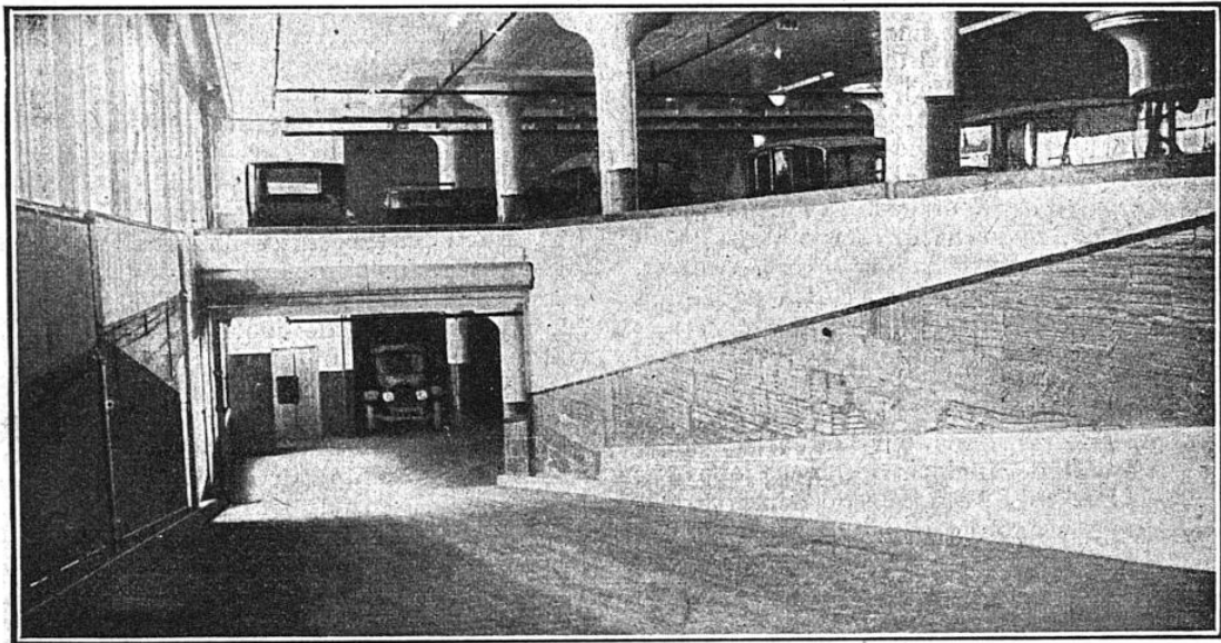
ON ACCÈDE AUX QUATRE ÉTAGES DE L'ÉTABLISSEMENT PAR DE LARGES RAMPES Ces rampes, en béton armé, évitent, aux heures d'affluence, la confusion qui se manifeste dans les garages, aux abords des monte-charges. Elles permettent à deux voitures de se croiser sans gêne.
