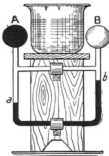
Si un vase d'eau chaude est placé à égale distance de deux boules réunies par un tube contenant du mercure, la boule A, noire et mate, absorbera beaucoup plus de chaleur que la boule dorée et polie B, et la différence entre les niveaux a et b accusera les degrés respectifs du pouvoir absorbant de A et de B.
