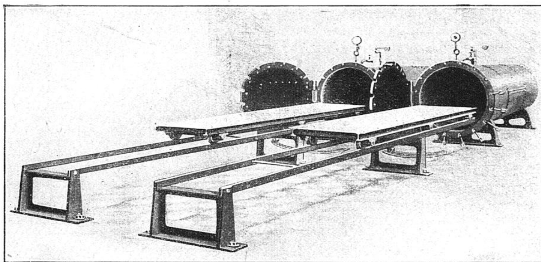
AUTOCLAVES HORIZONTAUX POUR LA VULCANISATION DES CHAMBRES A AIR
