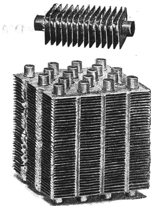
TUBES GARNIS D'AILETTES MÉTALLIQUES
