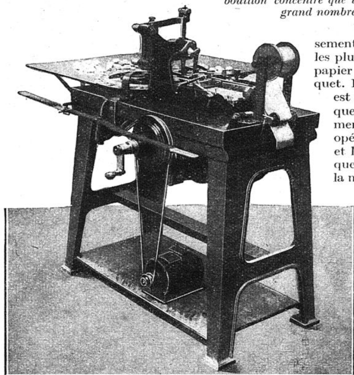
ENVELOPPAGE MÉCANIQUE DE CHOCOLATS PRALINÉS
