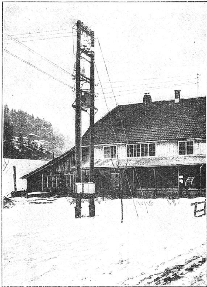
TRANSFORMATEUR A COURANT TRIPHASÉ, MONTÉ SUR POTEAUX, AVEC ISOLEMENT A L'HUILE
