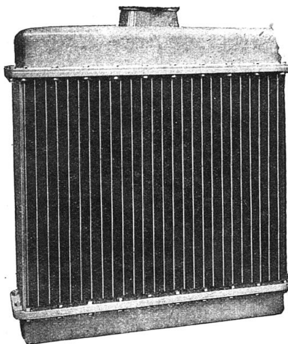
TYPE DE RADIATEUR POUR CAMION Lourd Les collecteurs d'eau sont boulonnés au-dessus et au-dessous du bloc de tubes du radiateur.
