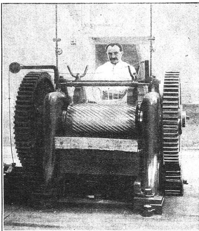
MACHINE A DÉCHIUQUETER LE CAOUTCHOUC BRUT Entre deux cylindres à grosses cannelures et sous un courant d'eau froide, les boules de caoutchouc sont broyées et agglomérées.
