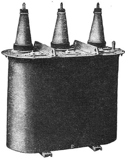
TRANSFORMATEUR TRIPHASÉ On remarquera avec quel soin les bornes sont isolées.
