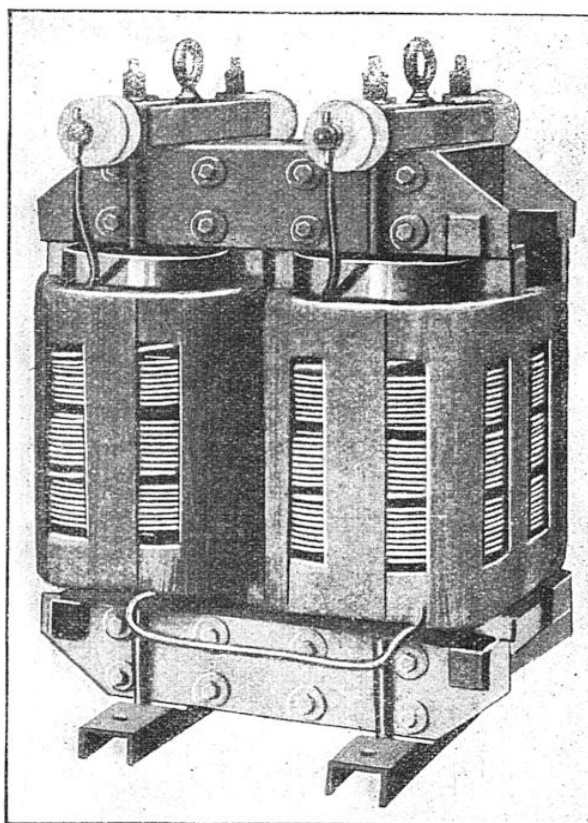
TRANSFORMATEUR MONOPHASÉ POUR FAIBLES PUISSANCES
