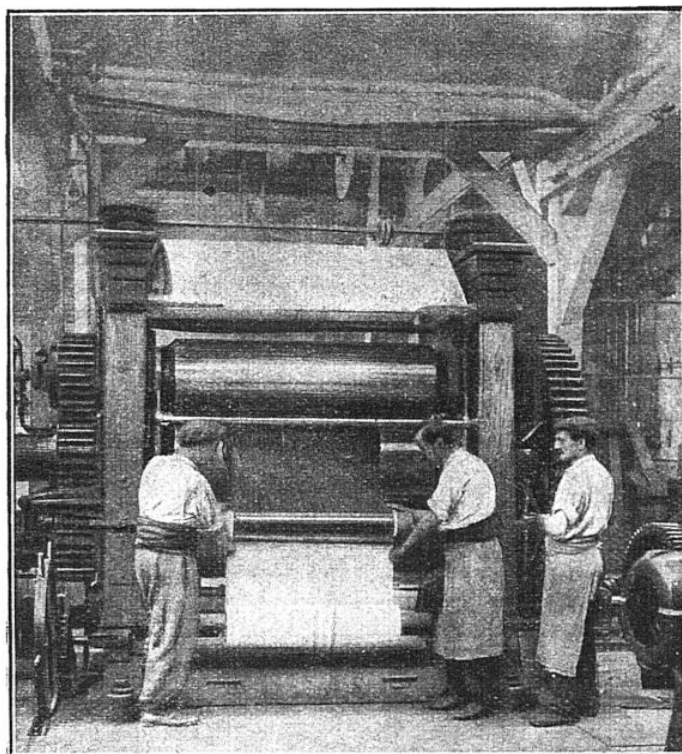
LE MÉLANGE DE CAOUTCHOUC PASSÉ A LA CALANDRE Les feuilles laminées sont recueillies entre des toiles afin d'éviter qu'elles ne se soudent les unes aux autres.
