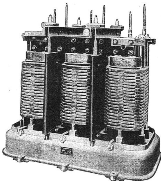
TRANSFORMATEUR TRIPHASÉ, A VENTILATION FORCÉE, POUR GRANDES PUISSANCES
