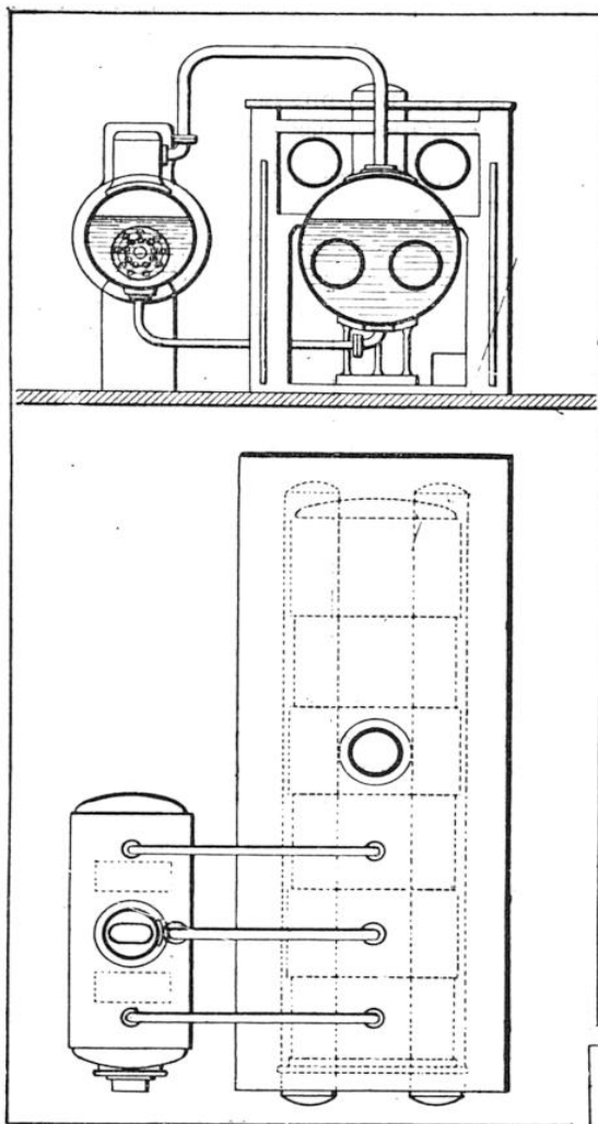
CHAUDIÈRE ÉLECTRIQUE DE 500 KILOWATTS, ACCOUPÉE AVEC UNE CHAUDIÈRE A CHARBON EXISTANTE
