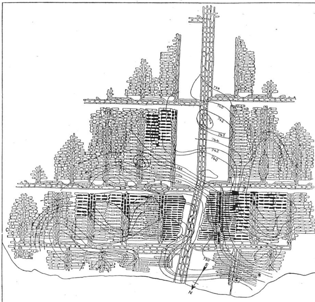
PLAN DE L'EXPLOITATION SOUTERRAINE D'UNE MINE DE HOUILLE AMÉRICAINE
