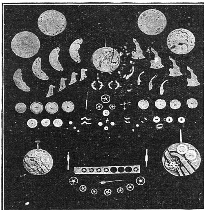
PARTIES CONSTITUTIVES DU MOUVEMENT DES MONTRES DANS L'ORDRE DE FABRICATION
