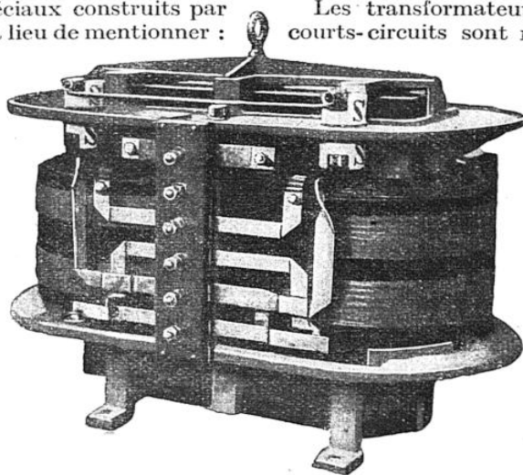
TRANSFORMATEUR MONOPHASÉ, RÉGLABLE, POUR LA SOUDURE AUTOGÈNE
