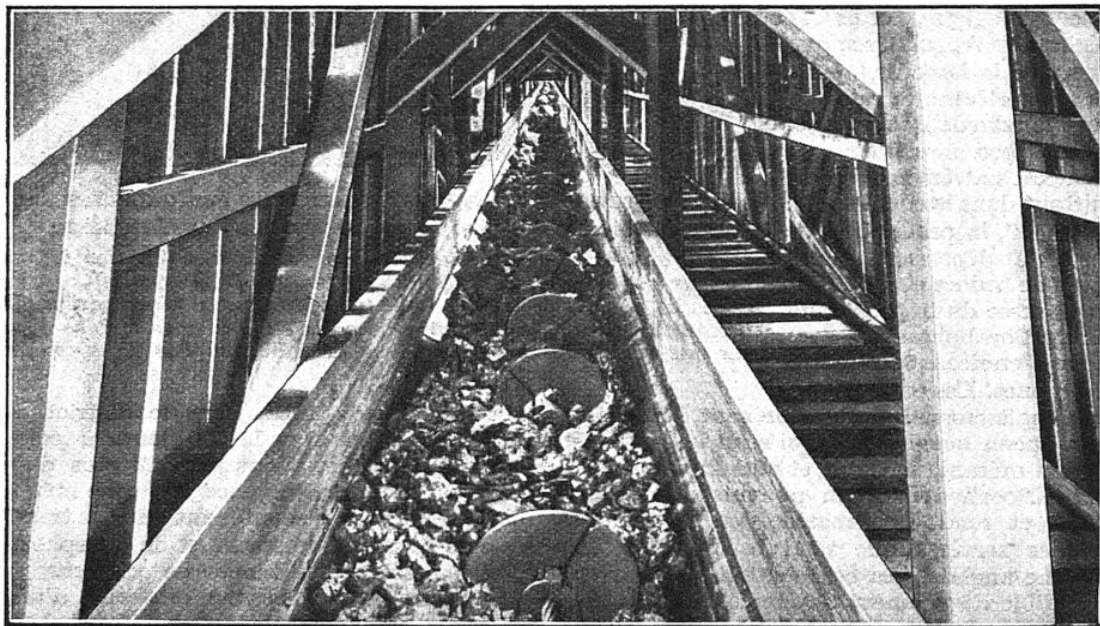
VUE D'UN CONVOYEUR A HOUILLE MU MÉCANIQUEMENT PAR L'ÉLECTRICITÉ
