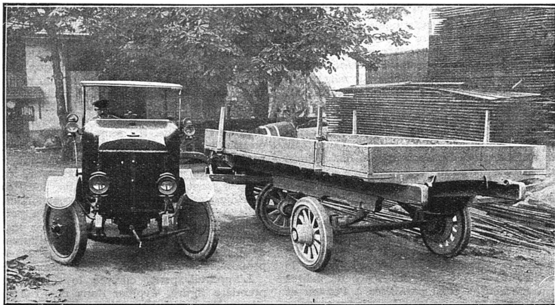
LE TRACTEUR ET LA REMORQUE PEUVENT ÉVOLUER DANS UN ESPACE TRÈS RESTREINT L'avant-train de la remorque est monté sur cheville ouvrière; d'autre part, l'attache du tracteur pouvant tourner complètement autour d'un axe rigide, il s'ensuit que le train peut se mouvoir dans un espace à peine plus large que les deux véhicules accolés.
