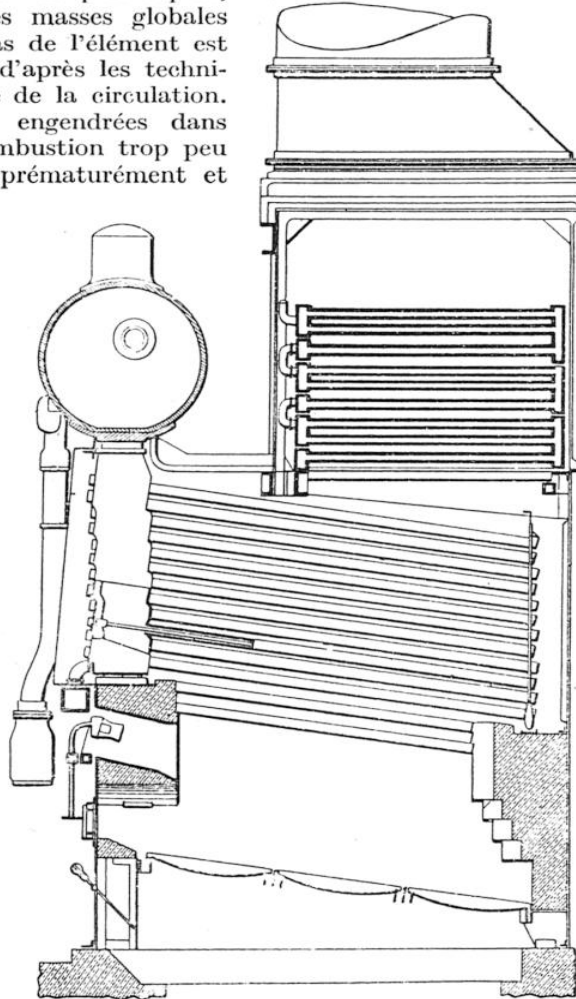
COUPE VERTICALE DE LA CHAUDIÈRE NICLAUSSE L'ensemble du faisceau tubulaire est divisé en deux parties : le faisceau inférieur et le faisceau supérieur, comme le montre la figure.
