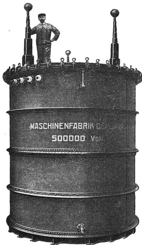
TRANSFORMATEUR D'ESSAIS DE 500.000 VOLTS PLONGÉ DANS SA CUVE À HUILE
