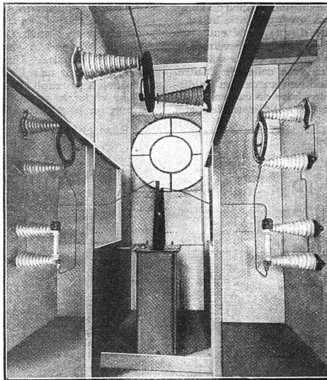
TRANSFORMATEUR DE MESURE, 65.000 VOLTS
