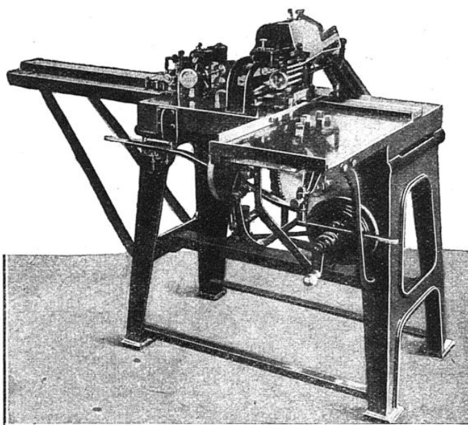
MACHINE UTILISÉE POUR FAIRE DES PAQUETS DE 3, 4, 5 CUBES ET MÊME D'AVANTAGE, JUSQU'À 10.
