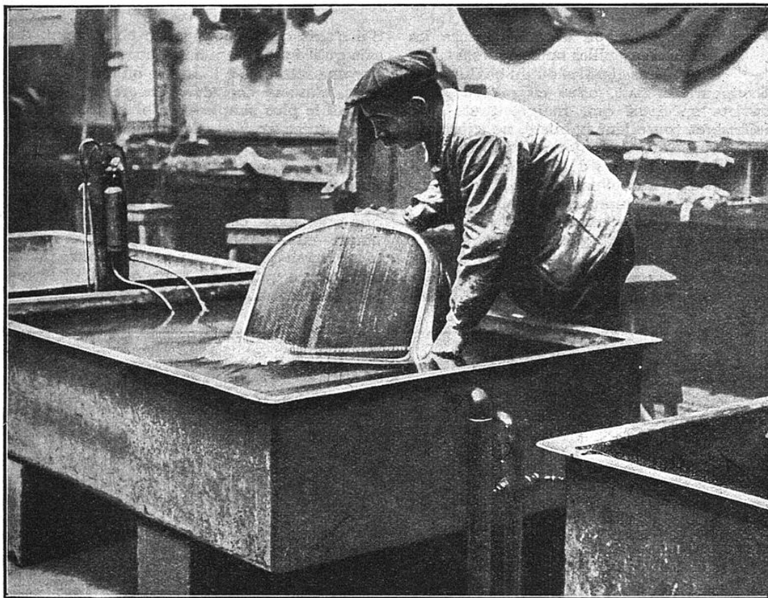
L'ESSAI DU RADIATEUR CONSTITUE L'OPÉRATION FINALE
