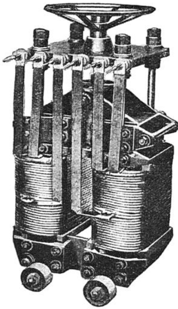
TRANSFORMATEUR DE 35.000 VOLTS, A BAIN D'HUILE
