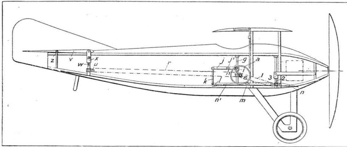
COUPE SCHÉMATIQUE D'UN AVION A INCIDENCE COMMANDÉE
