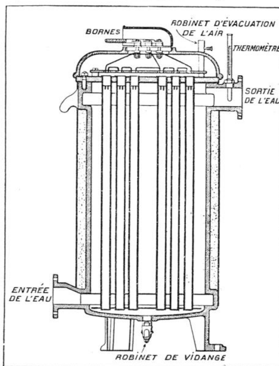
COUPE D'UNE CHAUDIÈRE ÉLECTRIQUE Dispositif de chauffage pour eau courante.
