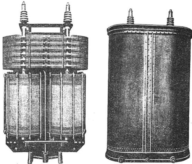
TRANSFORMATEUR MONOPHASÉ DE 2.400 KILOWATTS
