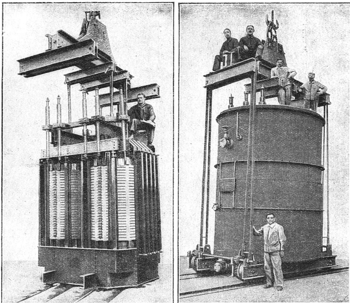
TRANSFORMATEUR DE 65.000 VOLTS (A GAUCHE) ET SA CUVE (A DROITE)
