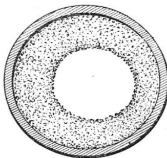
FAC-SIMILÉ, EN VRAIE GRANDEUR, D'UNE COUPE OBTENUE A LA SCIE DANS UN TUBE A CIRCULATION TRÈS ACTIVE. On y voit un dépôt d'environ un centimètre d'épaisseur.
