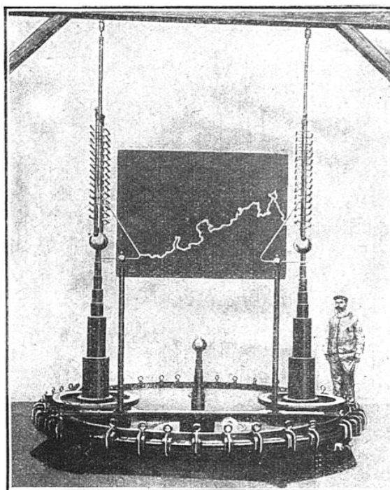
LE TRANSFORMATEUR D'ESSAIS DE 500.000 VOLTS EN FONCTIONNEMENT
