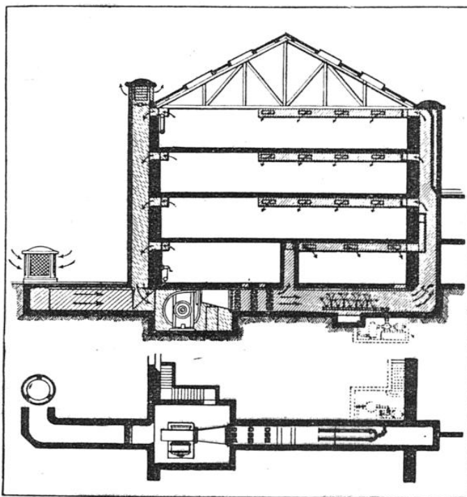
SCHÉMA D'UNE DISTRIBUTION DE CHAUFFAGE ÉLEC- TRIQUE DANS UNE IMPORTANTE FILATURE
