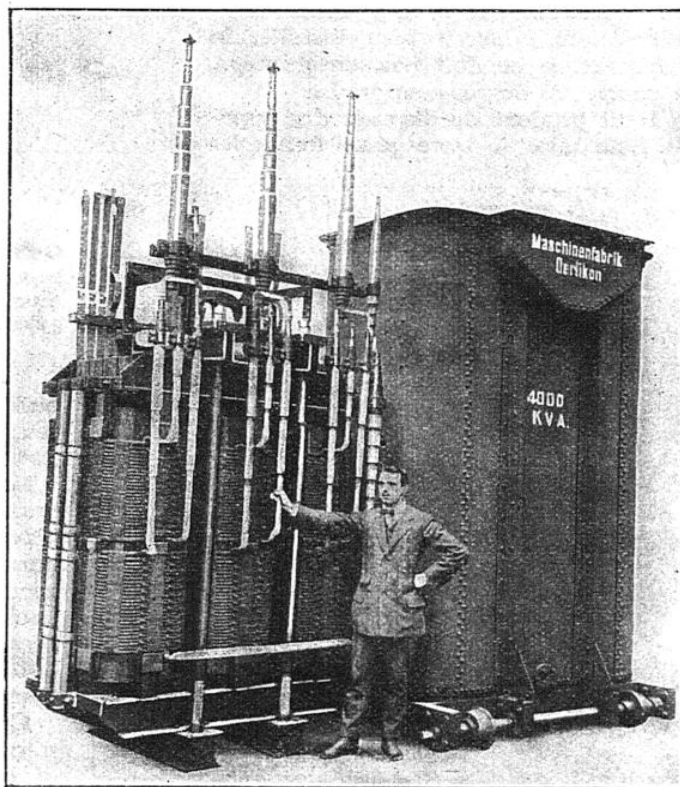
TRANSFORMATEUR TRIPHASÉ DE 4.000 KILOWATTS, 65.000 VOLTS, A BAIN D'HUILE
