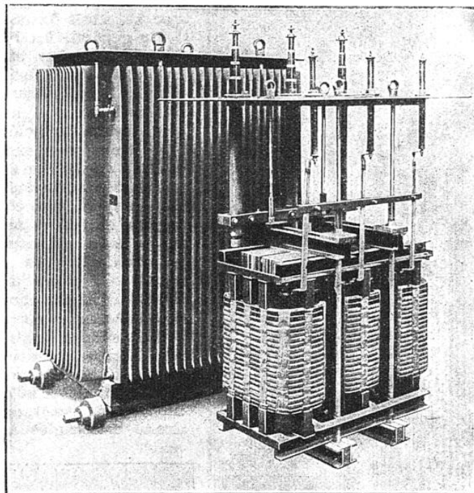
TRANSFORMATEUR TRIPHASÉ, A BAIN D'HUILE, A REFROIDISSEMENT PAR CIRCULATION D'EAU
