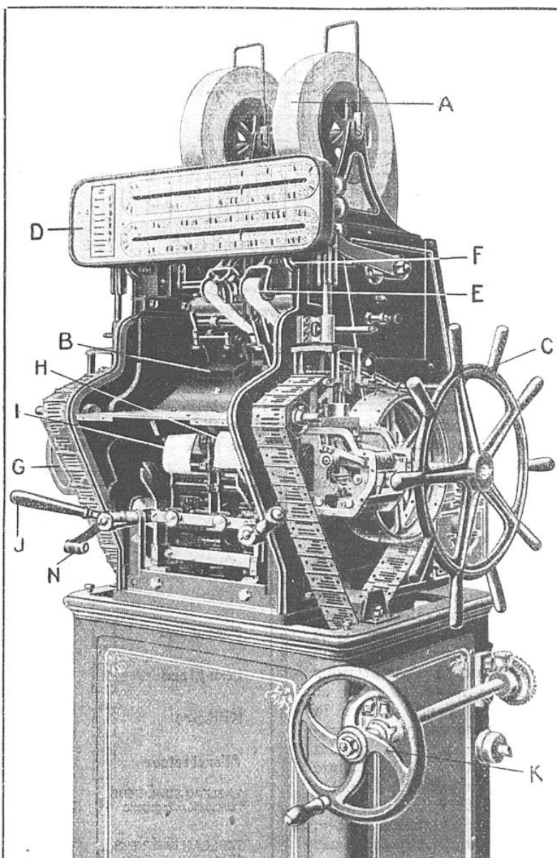
VUE DE FACE DU MÉCANISME DE L'APPAREIL CONTRÔLEUR FABRICANT LES BILLETS DE CHEMINS DE FER AUTOMATIQUEMENT A, bande de carton ; B, orifice de sortie du billet terminé ; C, cabestan ; D, tableau de distribution ; E, feuille de contrôle ; F, totalisateur général ; G, additionneur ; H, tambour ; I, feuille de récapitulation ; J, manette ; N, levier d'embrayage ; K, volant.
