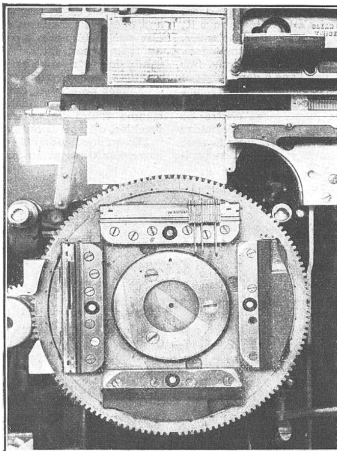
ROUE-MOULE DE LINOTYPE A MOULES MULTIPLES
