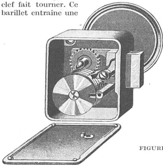
VUE INTÉRIEURE D'UNE SERRURE YALE MONTRANT LES DISQUES DES COMBINAISONS, ENTRAÎNÉS ICI PAR L'INTERMÉDIAIRE DE PETITS PIGNONS DENTÉS
