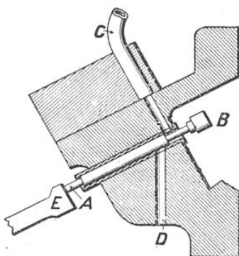
FIG. 13. — COUPE D'UNE VALVE DE DISTRIBUTION D'AIR COMPRIMÉ
