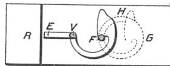
FIG. 14. — FIGURE EXPLIQUANT L'ENTRAÎNEMENT DU VERROU R PAR LA VIS F, SOLIDAIRE DU BARILLET
