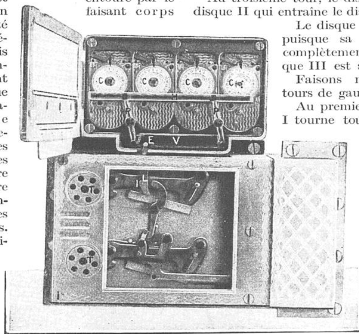
FIG. 31. — COMMANDE D'UNE PORTE DE COFFRE PAR LA SERRURE YALE A QUATRE COMBINAISONS
