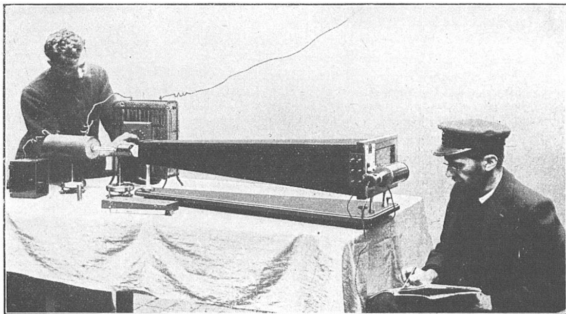
LE DILATOMÈTRE ENREGISTREUR CHEVENARD EN FONCTIONNEMENT
