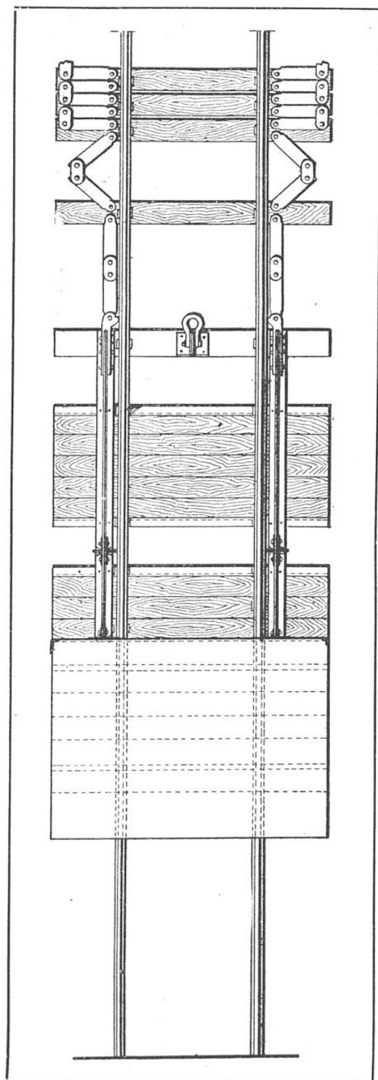
VUE EN PLAN DE LA VOIE, MONTRANT LE SYSTÈME DES TRAVERSES JOINTES L'UNE A L'AUTRE PAR DES TIGES ARTICULÉES Ces tiges permettent aux traverses de se déplacer plus ou moins, en formant frein-sabot, selon le recul du heurtoir, qui les entraîne avec lui au moyen des rails mobiles ou longrines quand il reçoit le choc violent d'un train ou de véhicules isolés.
