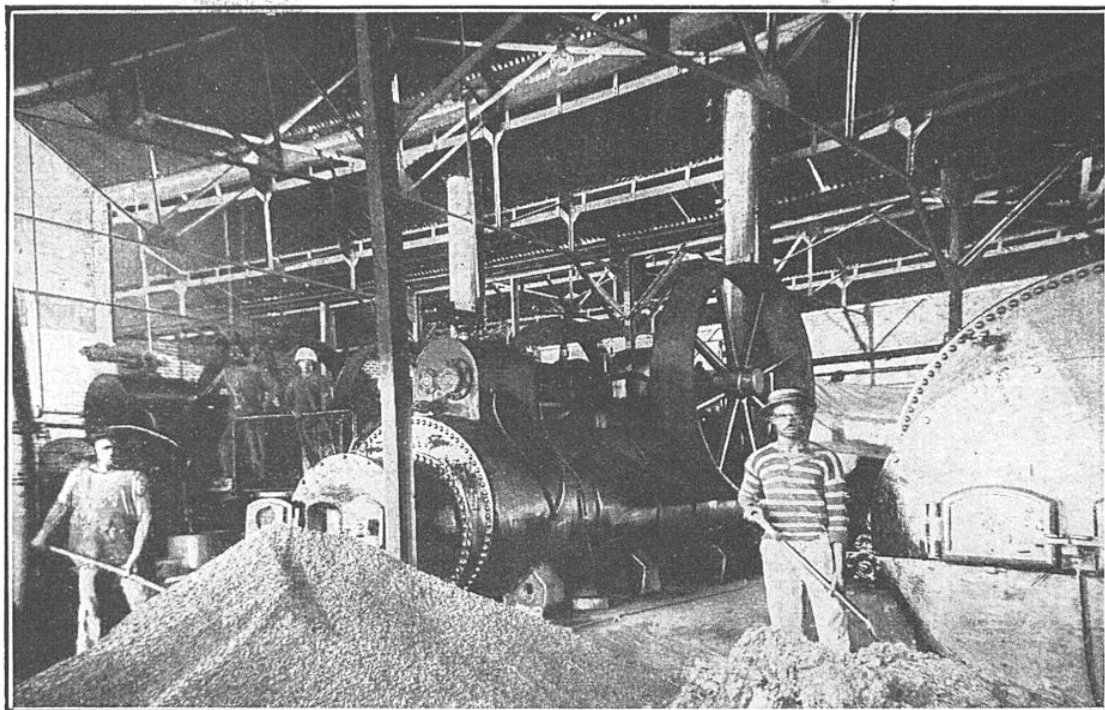
LES GÉNÉRATEURS D'UNE USINE A HUILE DE PALME, SUR LA CÔTE D'IVOIRE
