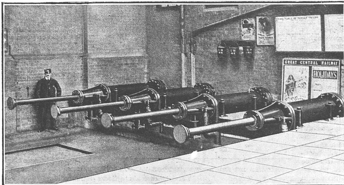
QUATRE HEURTOIRS HYDRAULIQUES, POUR DEUX VOIES PARALLÈLES, INSTALLÉS DANS UNE IMPORTANTE GARE ANGLAISE DU « GREAT CENTRAL RAILWAY »
