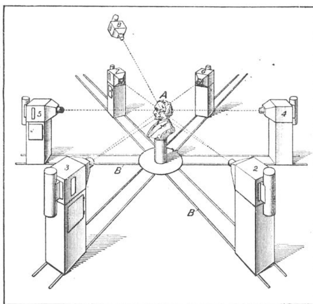
FIG. 1. — VUE EN PERSPECTIVE MONTRANT LE SYSTÈME OPTIQUE EMPLOYÉ
