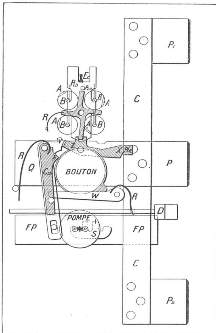
FIG. 18. — SERRURE DE COFFRE-FORT BAUCHE DANS SA POSITION DE FERMETURE
