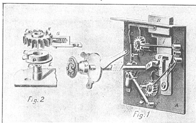
FIG. 9. — SERRURE A COMBINAISONS FICHET
