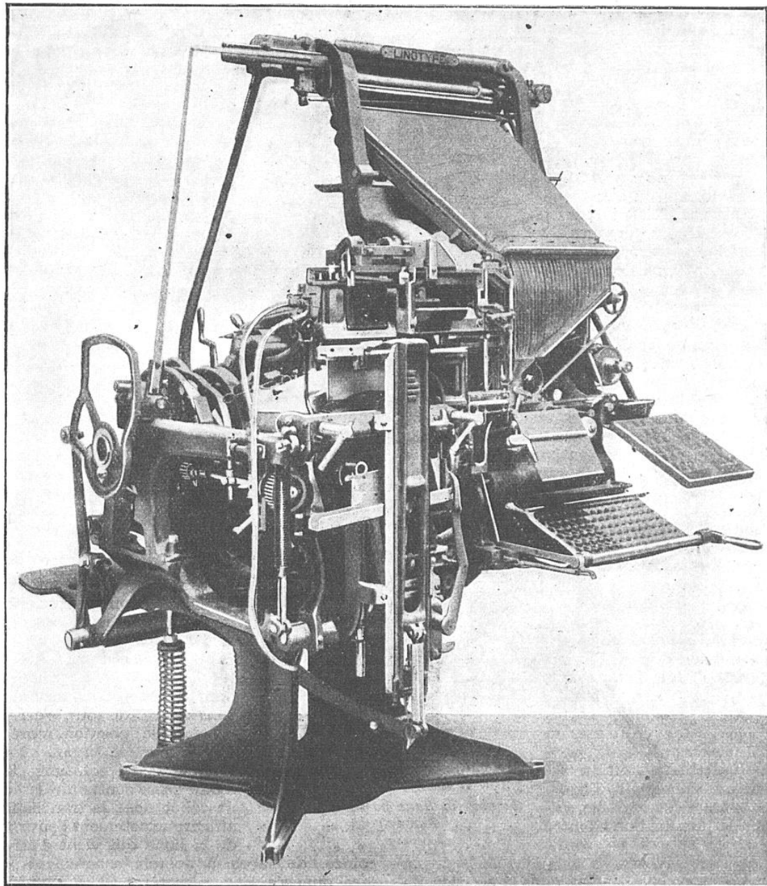
VUE D'AVANT D'UNE MACHINE LINO TYPE A UN SEUL MAGASIN (MODÈLE ANCIEN)
