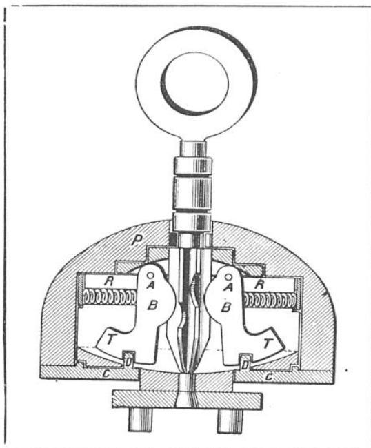
FIG. 20. — LE PLUS RÉCENT MODÈLE DES SERRURES SYSTÈME BAUCHE
