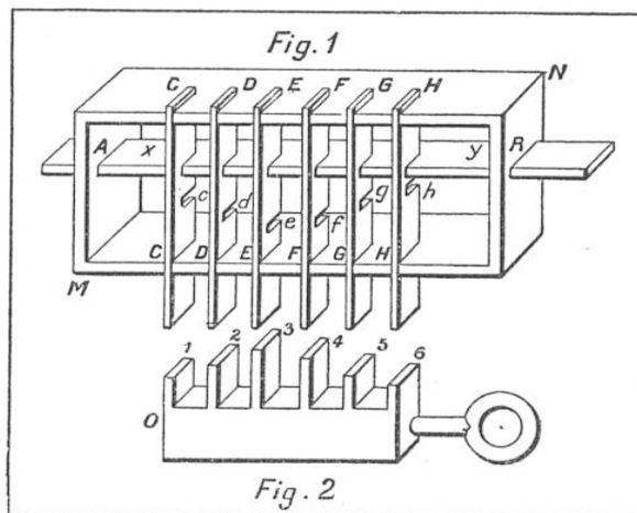
PLANCHE II. — PRINCIPE DE LA SERRURE DE SURETÉ DE JOSEPH BRAMAH
