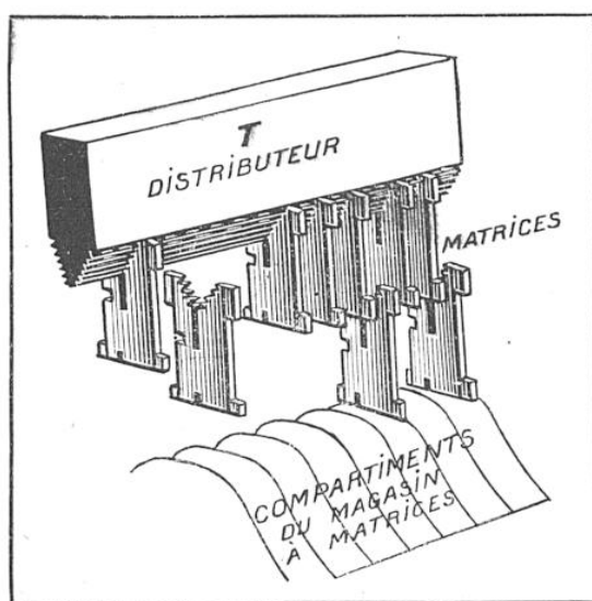
FIG. 8. — RETOUR DES MATRICES A LEURS PLACES NORMALES DANS LES COMPARTIMENTS DU MAGASIN DE LA LINOTYPE
