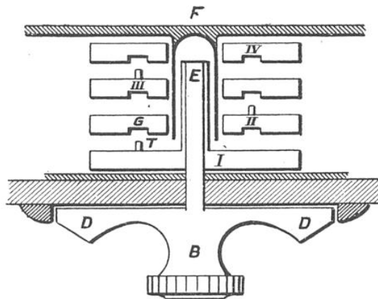
FIG. 30. — DESSIN SCHÉMATIQUE PERMETTANT DE COMPRENDRE LE MÉCANISME DES COMBINAISONS DANS LA SERRURE YALE
