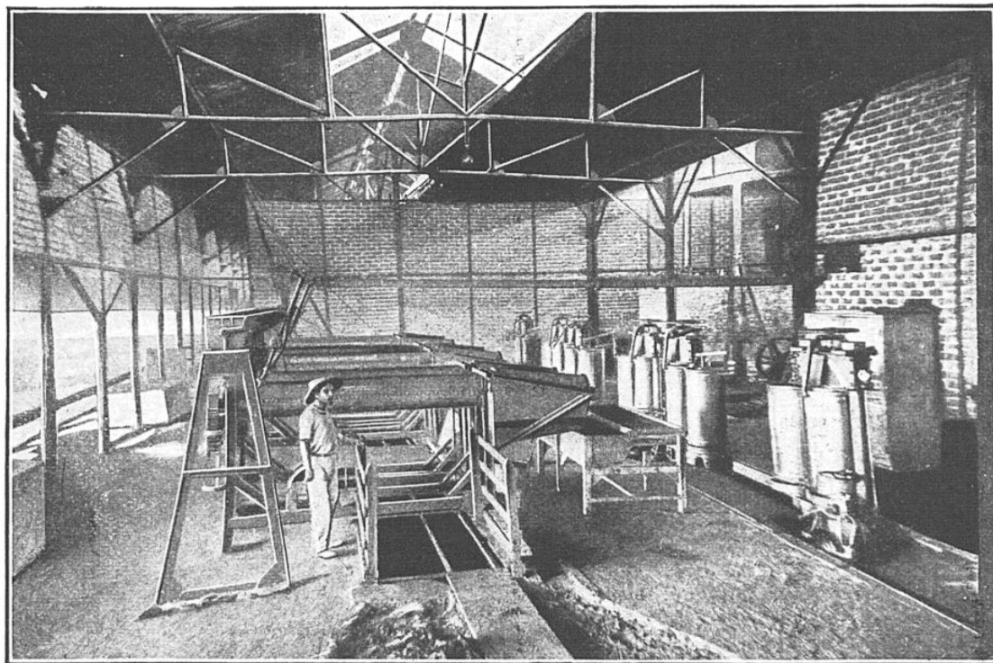
A GAUCHE : LES APPAREILS DITS RÉCHAUFFEURS ; A DROITE : LES PRESSES HYDRAULIQUES
