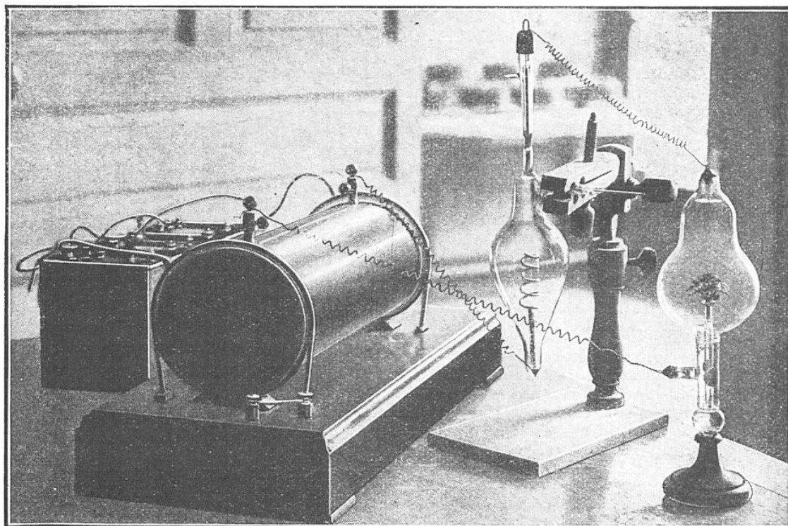
DISPOSITION DES APPAREILS POUR L'EXPÉRIENCE QUE MONTRE NOTRE FRONTISPICE Les fleurs du bouquet ne se distinguent alors que par leur forme; elles n'ont aucune couleur.
