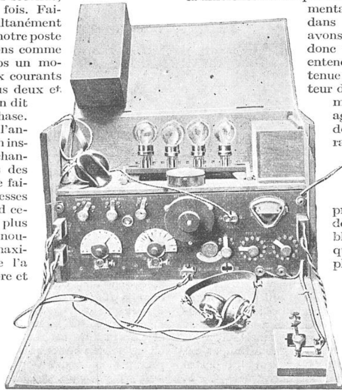
POSTE ÉMETTEUR ET RÉCEPTEUR DONNANT 400 KILOMÈTRES DE PORTÉE AVEC UN MAT HAUT DE 24 MÈTRES C'est un tel poste qui reliait le maréchal Foch aux quartiers généraux des diverses armées alliées. On le transportait en camionnette.
