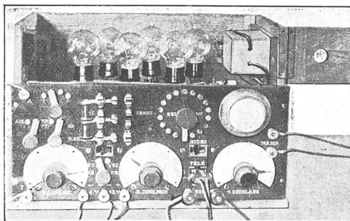
POSTE ÉMETTEUR ET RÉCEPTEUR EMPLOYÉ A TERRE, EN AVION ET SUR CHAR D'ASSAUT
