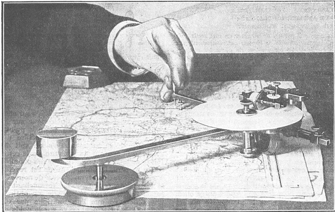
MODE D'EMPLOI DU PLANIMÈTRE POLAIRE A DISQUE TOURNANT POUR LE MESURAGE DE LA SUPERFICIE D'UN TERRAIN DONT ON POSSÈDE UN PLAN EXACT
