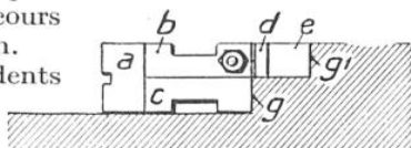
FIG. 27. — COUPE VERTICALE FAITE TRANSVERSALEMENT A L'ENSEMBLE DES COINS DE RÉGLAGE
