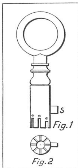
PLANCHE 13. - CLEF DE LA SERRURE BRAHMA S, panneton. La base de la clef porte des entailles dans lesquelles viennent se loger les lames de la figure 2 (planche de la page précédente).
