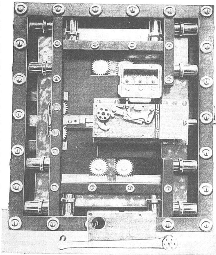
FIG. 33. — LA SERRURE D'UNE PORTE DE CHAMBRE-FORTE YALE, POSITION D'OUVERTURE
