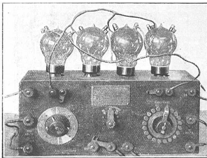
POSTE PUISSANT DOTÉ DE LAMPES A CORNES
