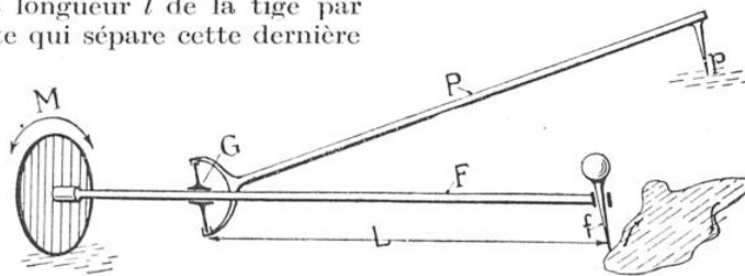
SCHÉMA INDICANT LE FONCTIONNEMENT D'UN PLANIMÈTRE DU SYSTÈME DIT POLAIRE
