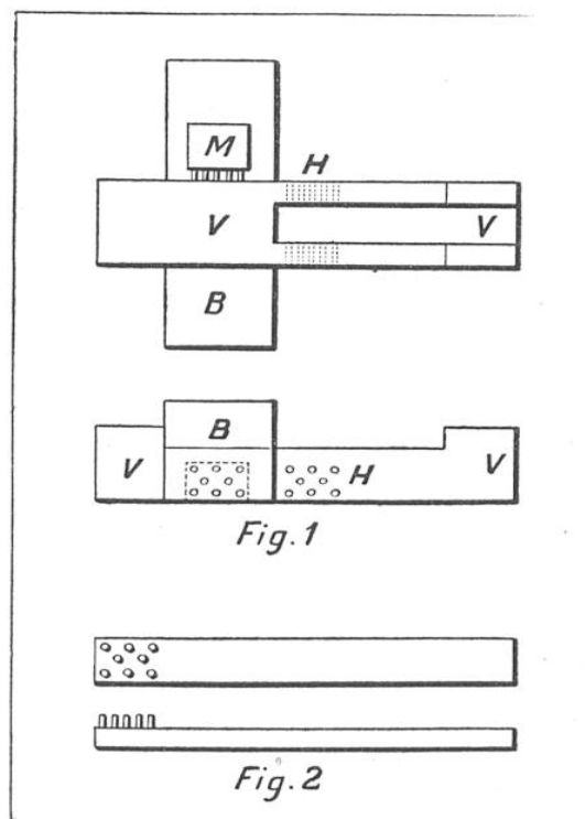
PLANCHE 10. — SERRURE ÉGYPTIENNE
