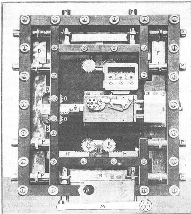
FIG. 32. — VUE DE LA SERRURE D'UNE PORTE DE CHAMBRE-FORTE YALE, POSITION FERMÉE
