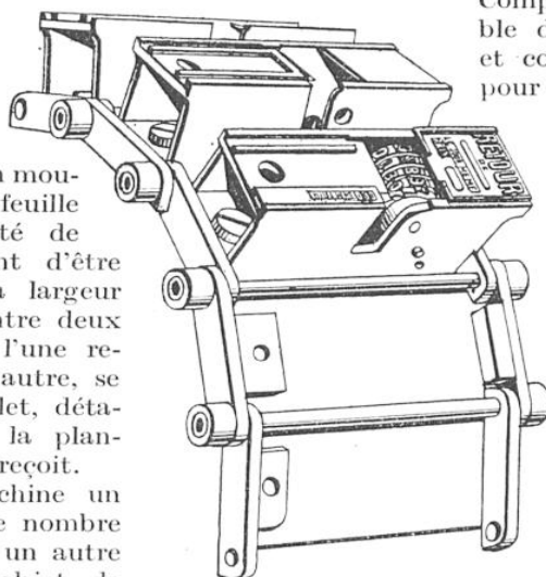
DISPOSITION DES COMPOSTEURS SUR LA CHAÎNE SANS FIN
