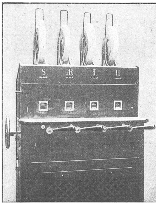
APPAREIL IMPRIMEUR-DISTRIBUTEUR DE TICKETS EN SERVICE DANS LES STATIONS DU MÉTRO
