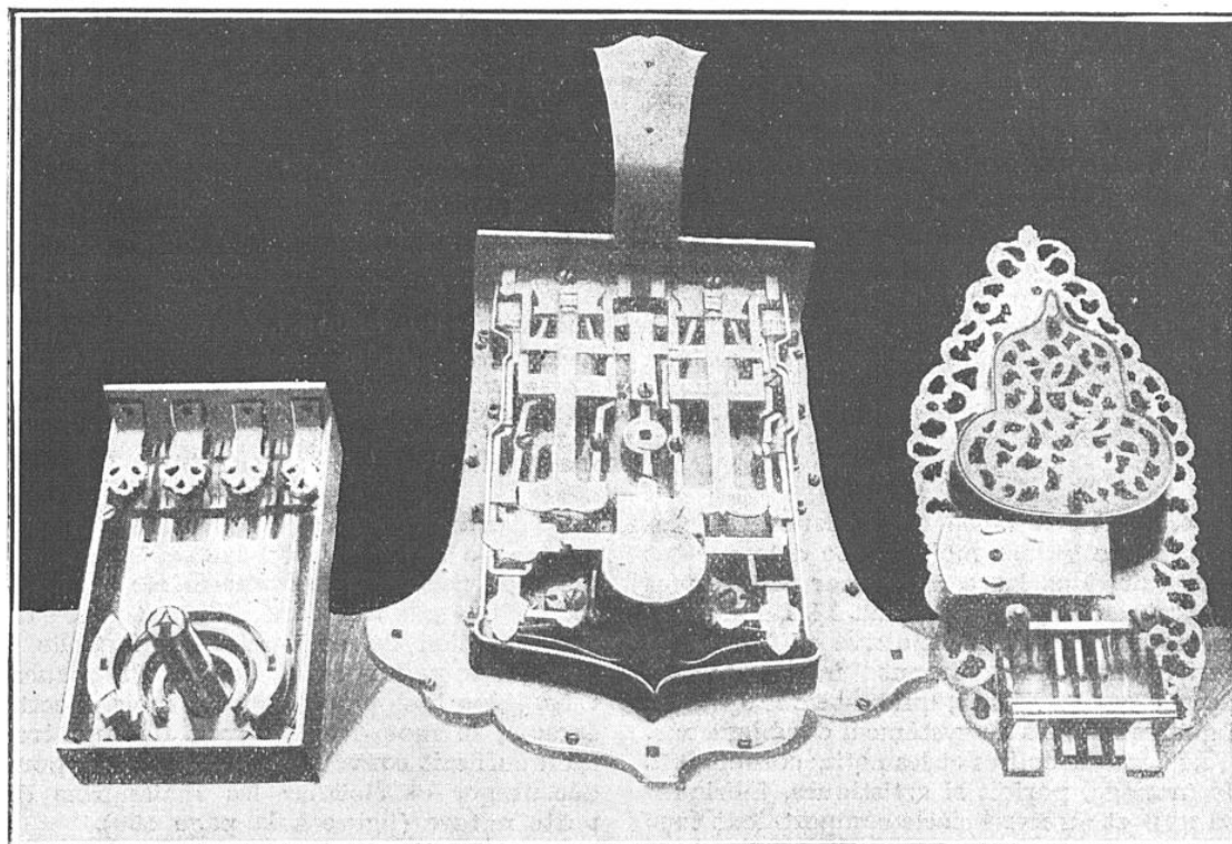
FIG. 6. — TROIS SERRURES ANCIENNES (COLLECTIONS DU MUSÉE DE CLUNY)
