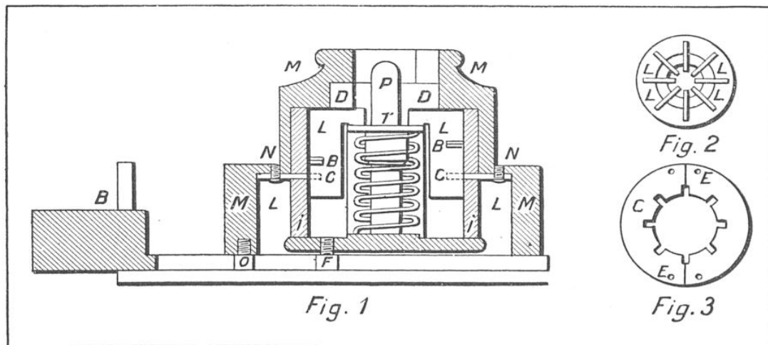
PLANCHE 12. — SERRURE JOSEPH BRAMAH, DITE SERRURE A POMPE
