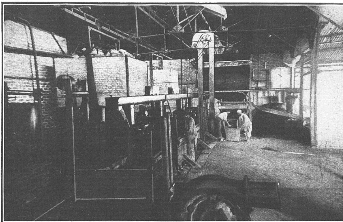
LE HALL DES APPAREILS DE CUISSON AVEC, AU FOND, LE CYLINDRE ROTATIF DANS LEQUEL SONT SÉCHÉES LES AMANDES CONTENANT L'HUILE PALMISTE
