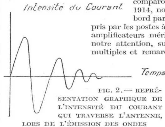
Ce courant, qui change très rapidement de sens, est amorti après une dizaine d'oscillations.
