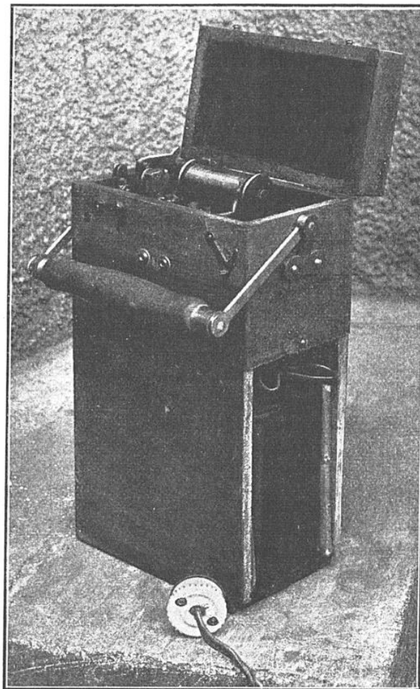
BOÎTE RENFERMANT L'ACCUMULATEUR OU LA PILE, LE CONDENSATEUR ET LE TREMBLEUR
