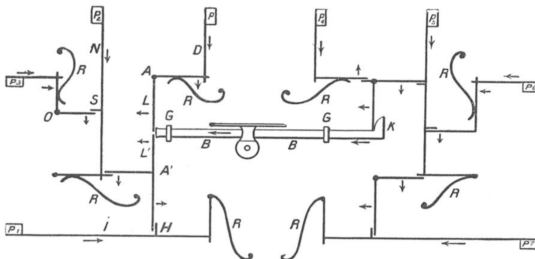
SCHÉMA DES PIÈCES ESSENTIELLES DE LA SERRURE DU COFFRE CI-DESSUS
