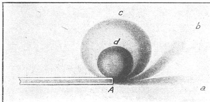
DANS UN CHAMP MAGNÉTIQUE UNIFORME, PERPENDICULAIRE A LEUR DIRECTION D'ÉMISSION, LES RAYONS CATHODIQUES S'ENROULENT SUR EUX-MÊMES
