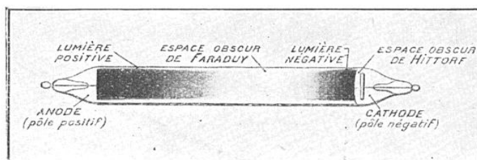
APPARENCE DE LA DÉCHARGE ÉLECTRIQUE DANS UN TUBE A GAZ RARÉFIÉ (PRESSION DE UN MILLIMÈTRE ENVIRON)
