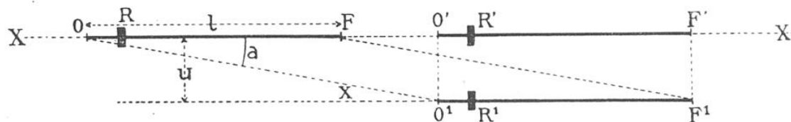
DÉMONSTRATION DE LA MANIÈRE DONT UNE DROITE OF , SE DÉPLAÇANT PARALLÈLEMENT A ELLE-MÊME, ENGENDRE LA SURFACE D'UN PARALLÉLOGRAMME OFF'O' DE BASE l ET DE HAUTEUR u , SURFACE ÉGALE A CELLE DU RECTANGLE O'F'O'1F'1 (VOIR DANS LE TEXTE, PAGE 482)
