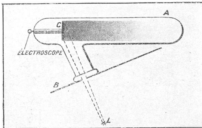
PRODUCTION DE RAYONS CATHODIQUES SOUS L'INFLUENCE DE LA LUMIÈRE ULTRA-VIOLETTE
