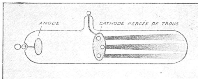
RAYONS-CANAUX ISSUS DES ORIFICES PERCÉS AU TRAVERS DE LA CATHODE DU TUBE
