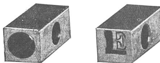
FIG. 10. — MATRICES DE MONOTYPES
