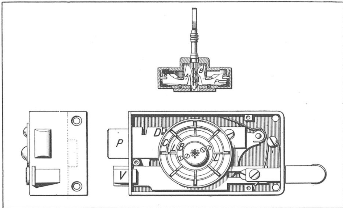
FIG. 17. — MODÈLE COURANT DES SERRURES SYSTÈME BAUCHE
