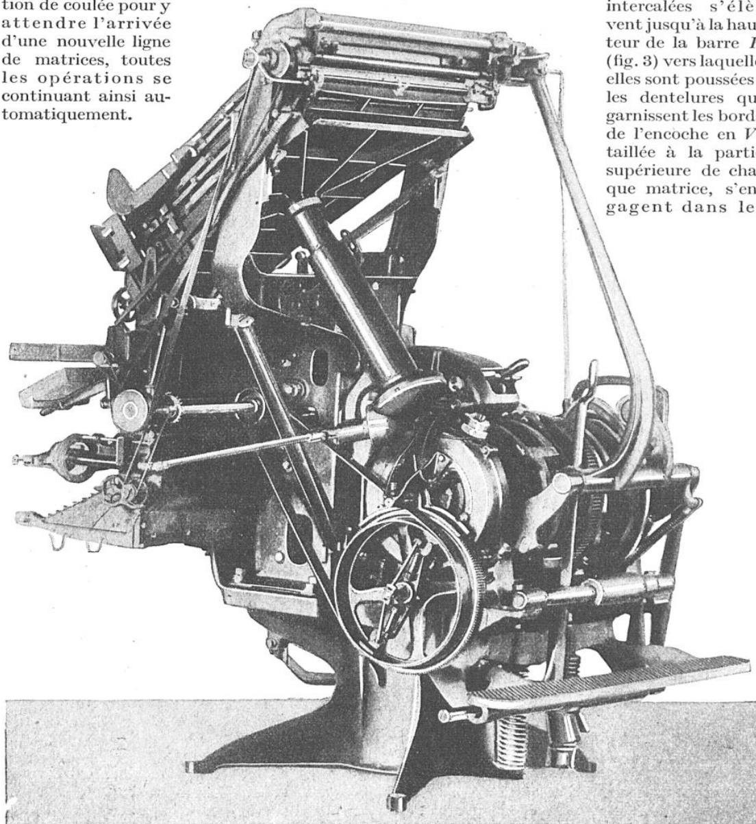
VUE D'ARRIÈRE D'UNE LINOTYPE A TROIS MAGASINS (MACHINE DE TYPE MODERNE)
