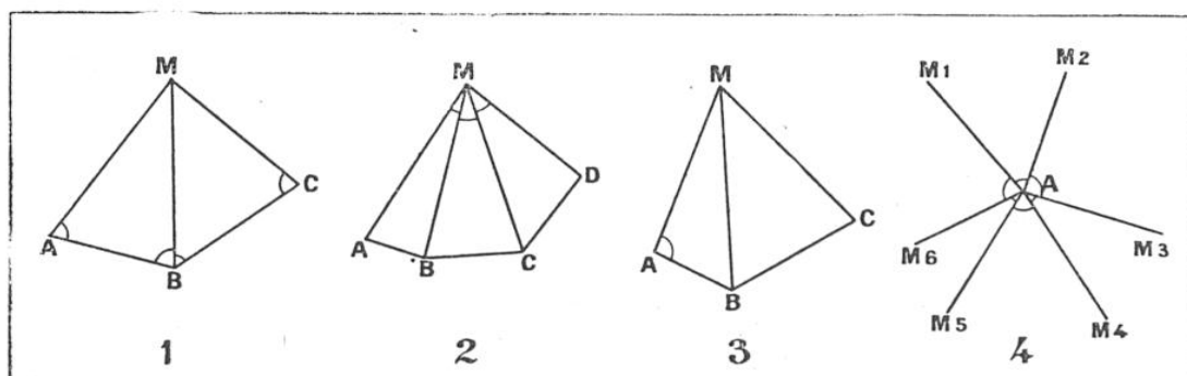
PLUSIEURS AUTRES MÉTHODES SONT EMPLOYÉES POUR LA DÉTERMINATION DE POINTS 1, par intersection ; 2, par relèvement ; 3, par recoupement ; 4, par rayonnement.
