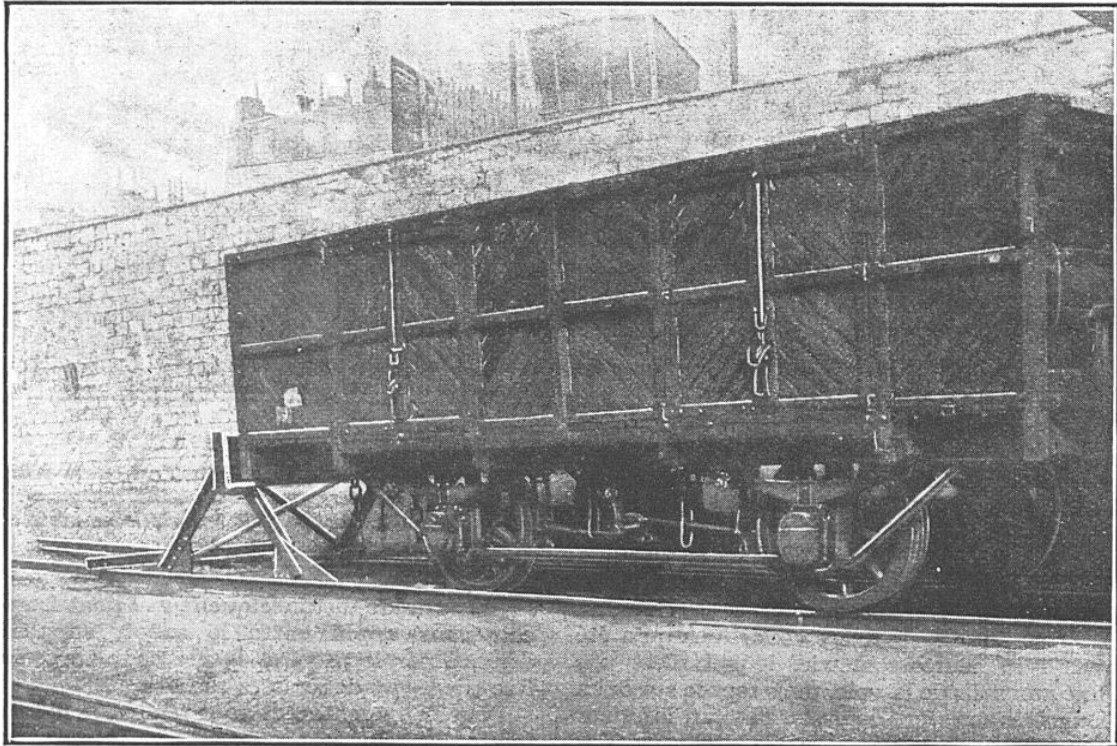
WAGON A MARCHANDISES ABORDANT LE HEURTOIR RAWIE
