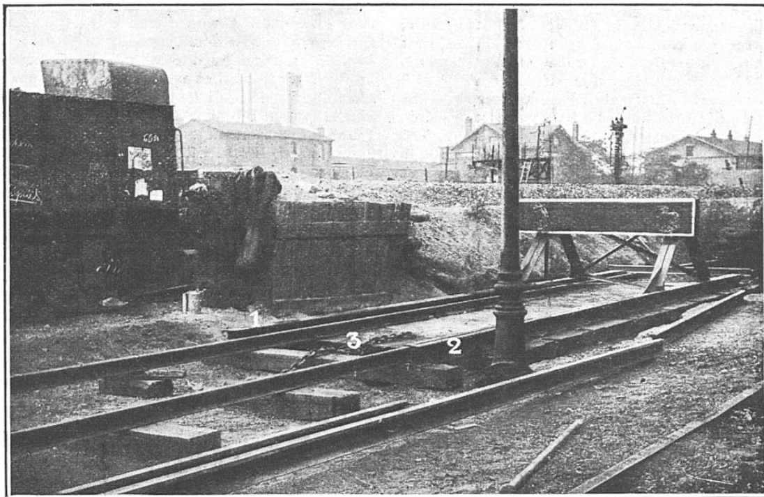
VUE GÉNÉRALE D'UN HEURTOIR GLISSANT A FREINAGE, SYSTÈME RAWIE
