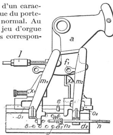
FIG. 21. — MÉCANISME DE MISE EN PLACE DU PORTE-MATRICES Ce mécanisme sert aussi au réglage de largeur des divers caractères et au réglage des espaces justificatives.
