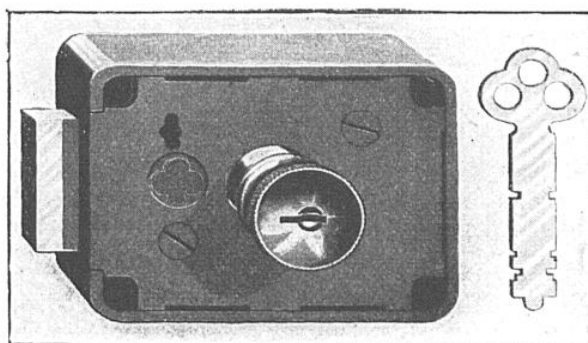
FIG. 24. — SERRURE YALE POUR APPARTEMENT On voit à droite un modèle de la clef spéciale Yale.
