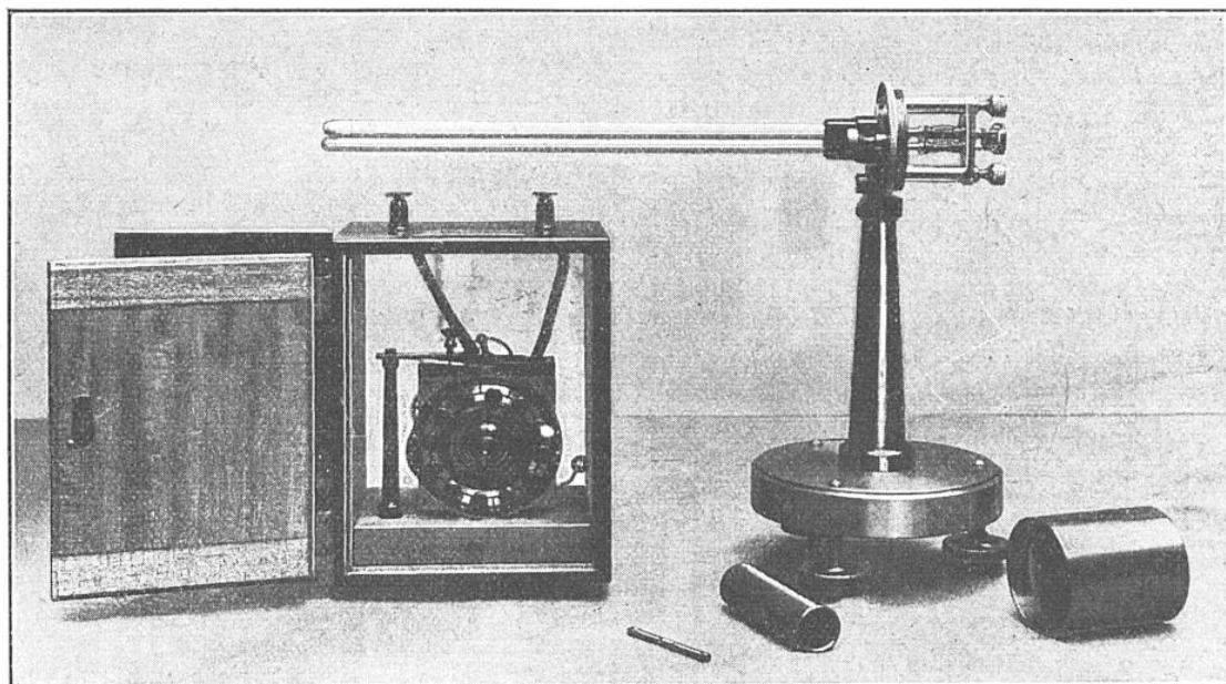
ORGANES DIVERS DU DILATOMÈTRE ENREGISTREUR DÉMONTÉ
