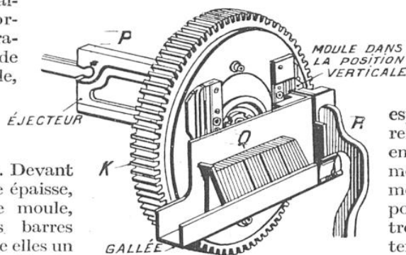
FIG. 6. — LA ROUE-MOULE EN POSITION D'ÉJECTION DE LA LIGNE
