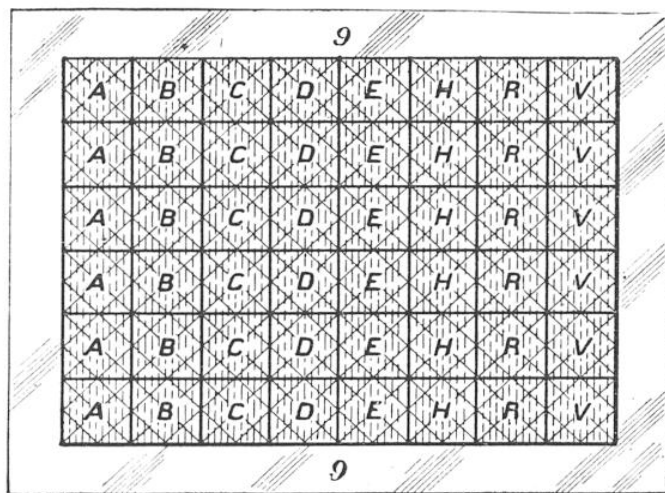
FIG. 2. — VUE EN PLAN DE L'UN DES ÉCRANS (9) AVEC SES LIGNES VERTICALES, HORIZONTALES ET OBLIQUES, CONTINUES ET INTERROMPUES, ET SES LETTRES DE REPÈRE DANS LES CARRÉS
