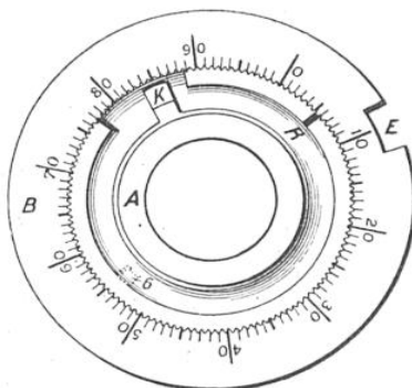
FIG. 27. — UN DISQUE DE COMBINAISON
