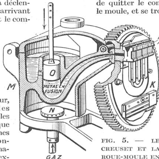
FIG. 5. — LE CREUSET ET LA ROUE-MOULE EN POSITION DE COULÉE, AVEC UNE LIGNE DE MATRICES EN PLACE
