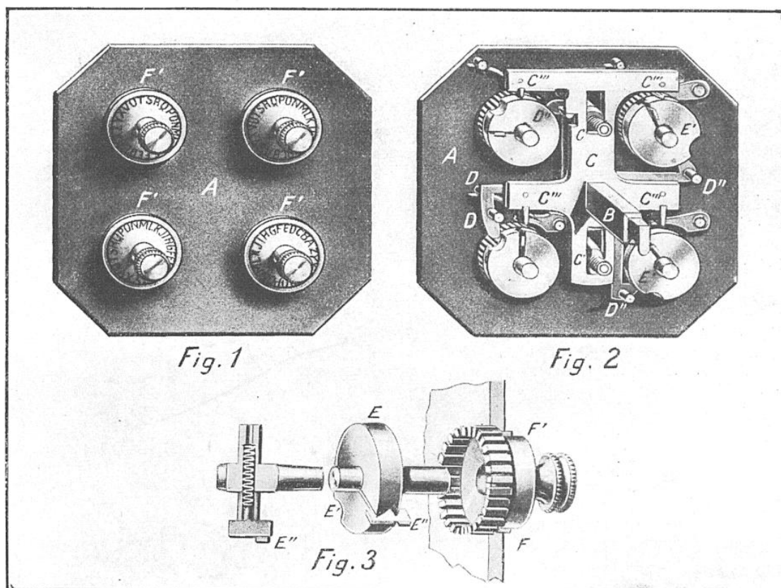
PLANCHE 8. — SERRURE A COMBINAISONS SYSTÈME DELARUE
