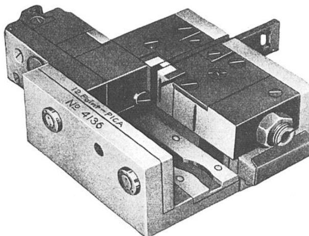
FIG. 24. — LE MOULE VU D'EN HAUT
