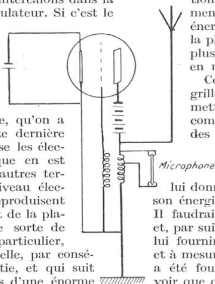
FIG. 10. — SCHÉMA D'UN POSTE ÉMETTEUR DE TÉLÉPHONIE SANS FIL
