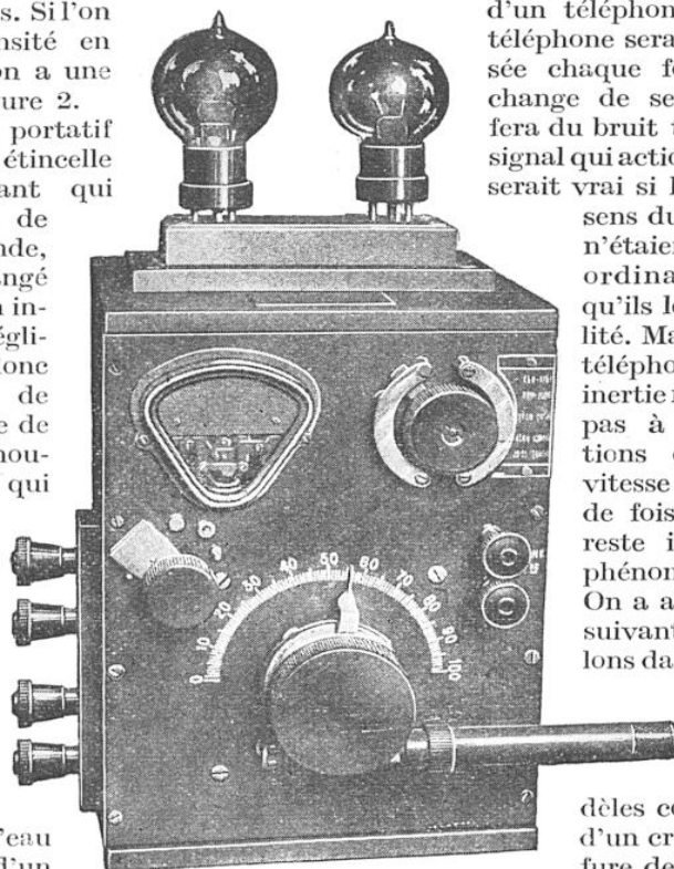
APPAREIL APPELÉ «HÉTÉRODYNE» C'est un générateur local d'ondes entretenues qui permet de recevoir les ondes, également entretenues, transmises, grâce au phénomène des battements.
