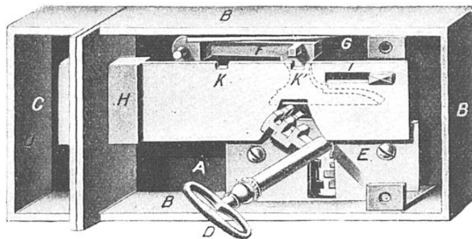
FIG. 1. — SERRURE ORDINAIRE A PÊNE DORMANT ET A UN TOUR
