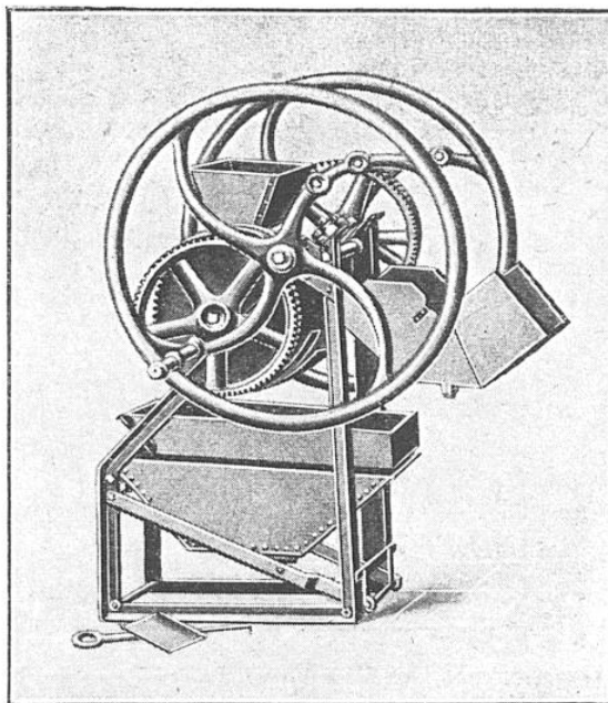
DÉPULPEUR A MAIN SYSTÈME HAAKE
