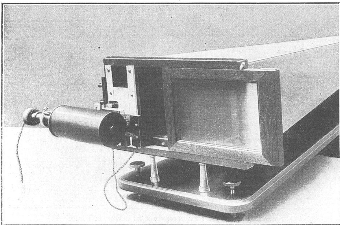
DISPOSITIF D'ÉCLAIRAGE DU DILATOMÈTRE ENREGISTREUR CHEVENARD
