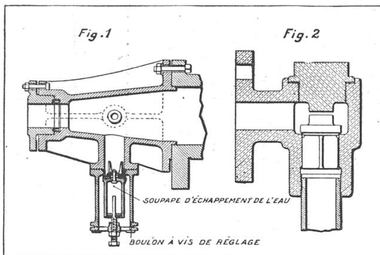
DÉTAILS DU FREIN HYDRAULIQUE RANSOMES ET RAPIERE
