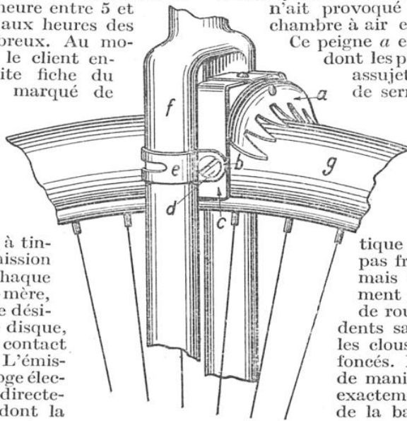
LE PEIGNE ARRACHE AU PASSAGE LES POINTES QUI S'ENFONCENT DANS LE PNEU
