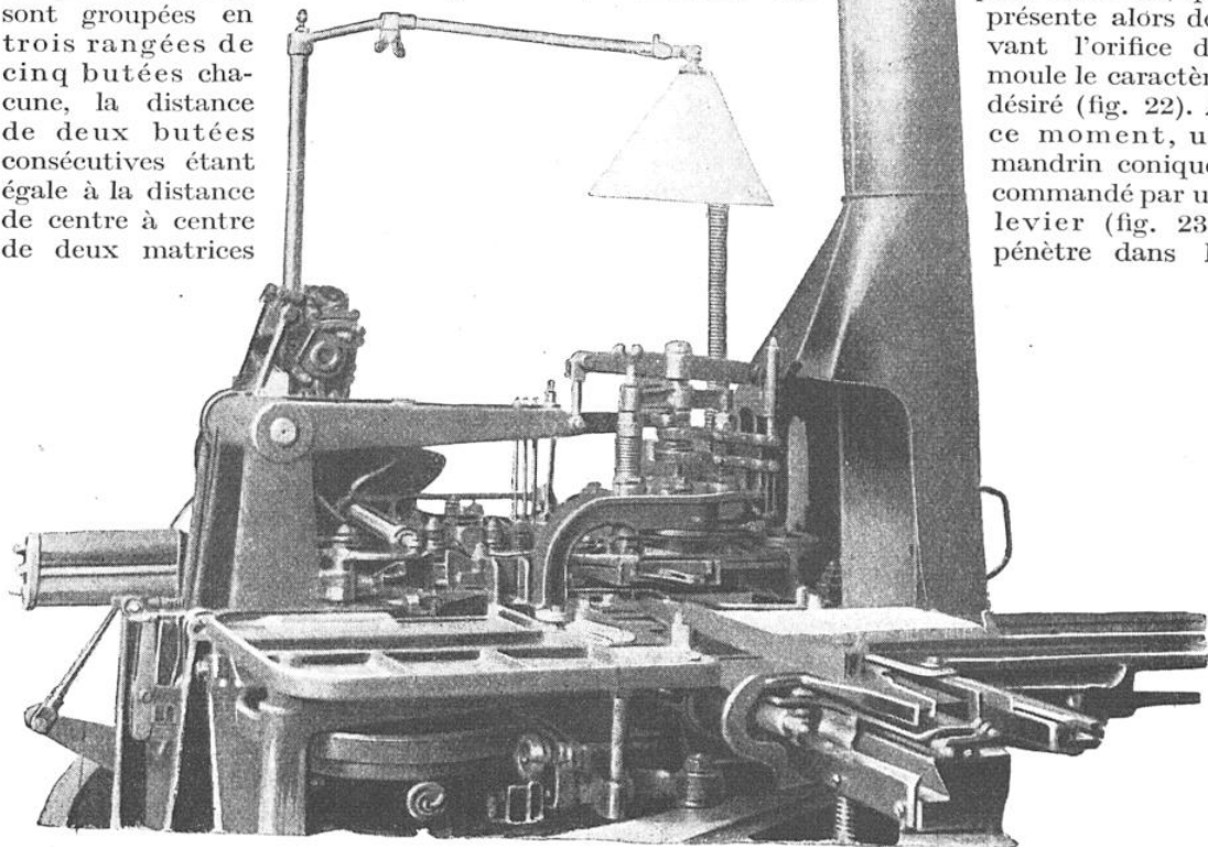
LES ORGANES ESSENTIELS, VUS EN ÉLEVATION, D'UNE FONDEUSE DE MACHINE MONOTYPE
