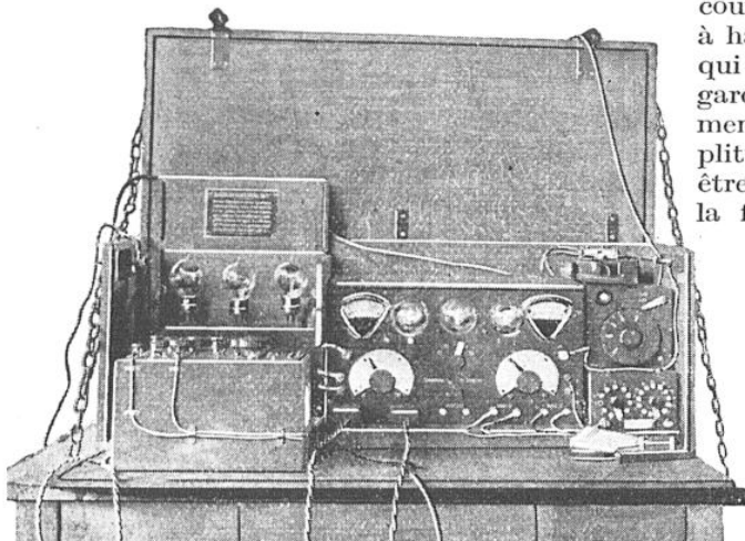
ENSEMBLE DU POSTE ÉMETTEUR ET RÉCEPTEUR TRANSPORTÉ EN CAMIONNETTE AUTOMOBILE
