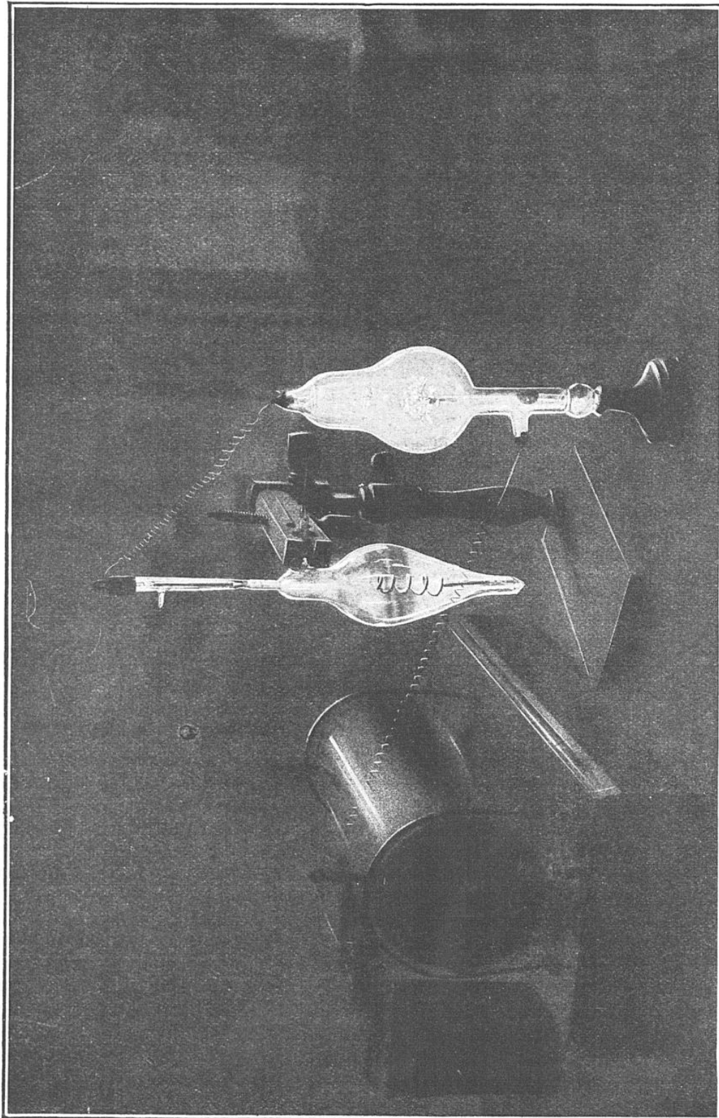
LE BOUQUET ARTIFICIEL, ET NORMALEMENT INCOLORE, RENFERMÉ DANS L'AMPOULE DROITE, REVÊT, SOUS L'INFLUENCE DES RAYONS CATHODIQUES, LES COULEURS LES PLUS DIVERSES ET LES PLUS BRILLANTES. CHAQUE FLEUR DE CE BOUQUET EST FAITE, EN EFFET, D'UNE MATIÈRE QUI PREND, LORSQUE SA PHOSPHORESCENCE EST EXCITÉE, UNE COLORATION PARTICULIÈRE
