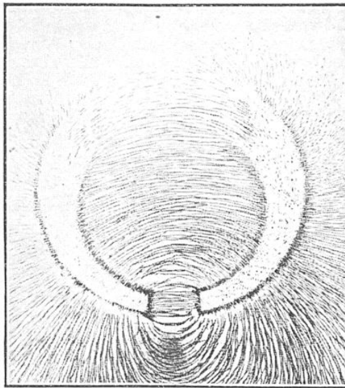
SPECTRE MAGNÉTIQUE D'UN AIMANT
