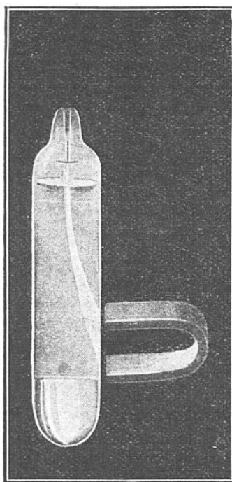
DÉVIATION D'UN FAISCEAU DE RAYONS CATHODIQUES PAR UN AIMANT
