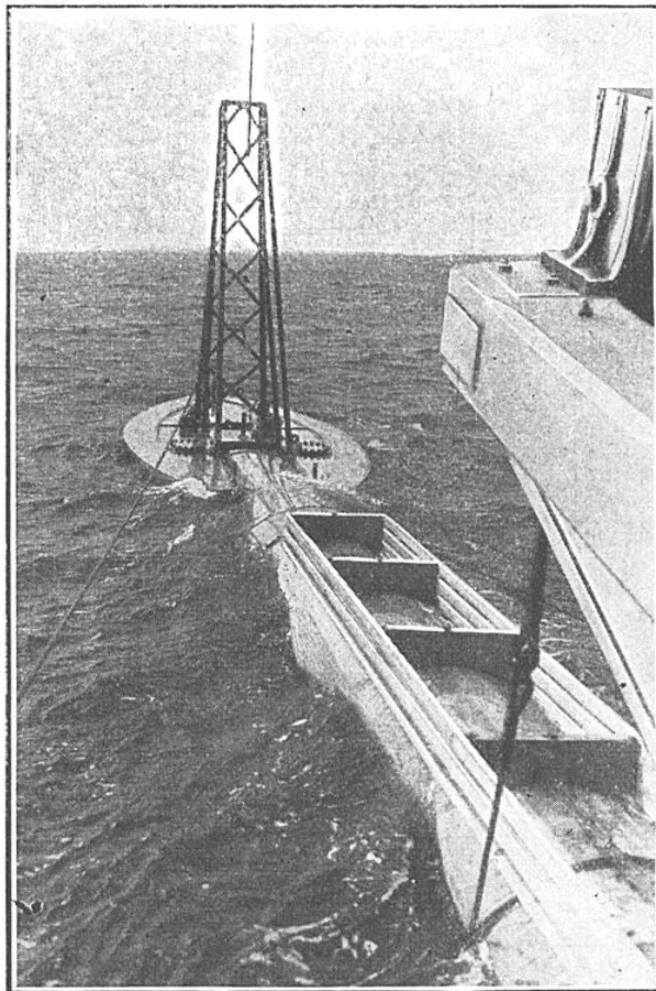
LE CAISSON SOUS-MARIN « ARGONAUT-III »
