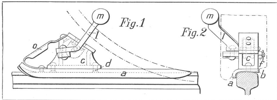
FREIN OU CALE-SABOT SUR LEQUEL EST ADAPTÉ UN DISPOSITIF ASSURANT SON RENVERSEMENT DÈS L'ARRÊT DU WAGON, LAISSANT ENSUITE LA VOIE LIBRE
