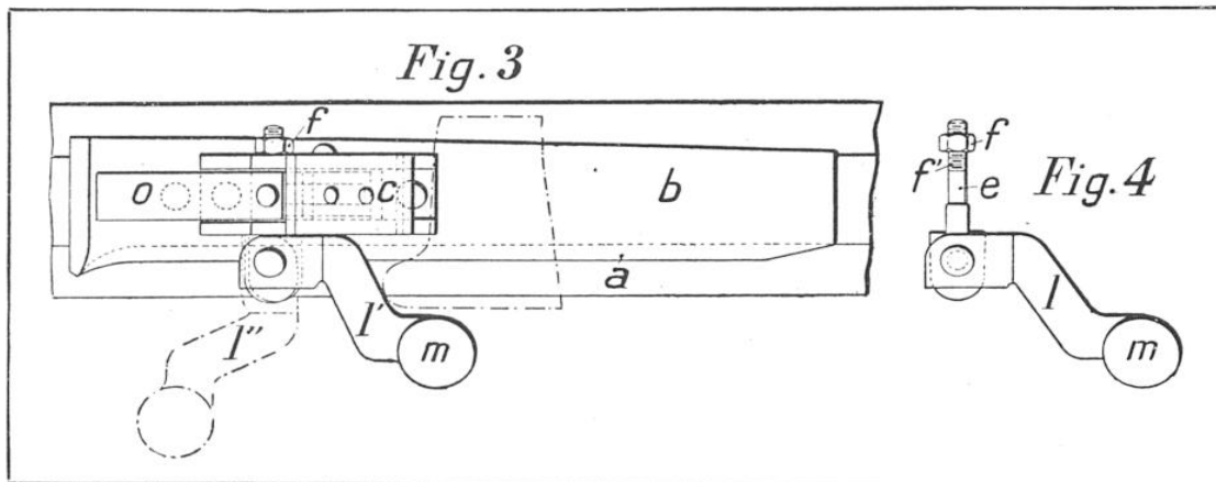
AUTRE ASPECT DU FREIN OU CALE-SABOT DE MM. GOUNON ET ROUCHET
