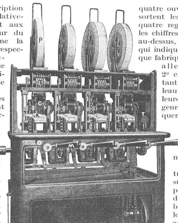
MÉCANISME DE L'APPAREIL IMPRIMEUR-DISTRIBUTEUR DE TICKETS
