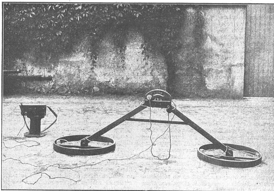
LA BALANCE D'INDUCTION « ALPHA », DU PROFESSEUR GUTTON, DE NANCY
