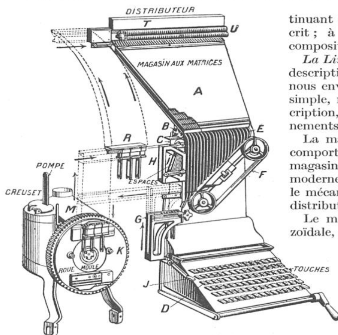
FIG. 3. — SCHÉMA D'ENSEMBLE D'UNE LINOTYPE
