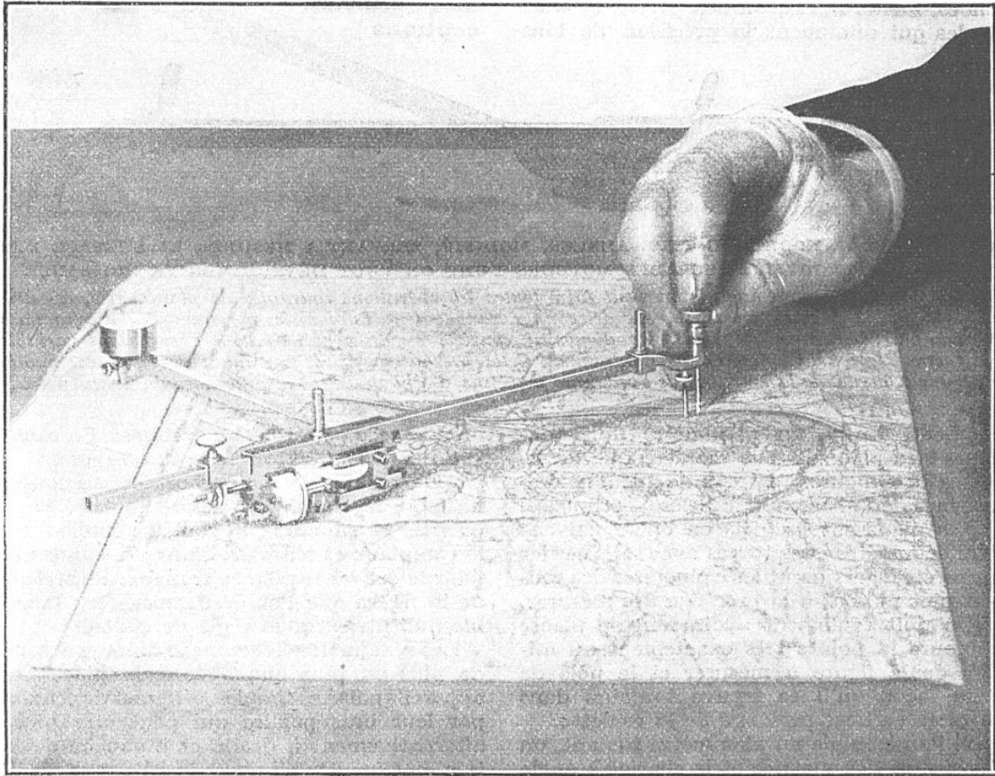
EMPLOI DU PLANIMÈTRE POLAIRE H. MORIN, DU TYPE AMSLER
