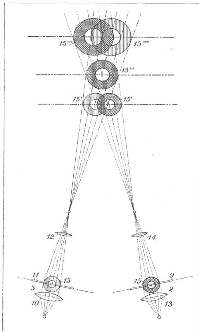
FIG. 5. — DIAGRAMME MONTRANT LE PRINCIPE ESSENTIEL DU PROCÉDÉ
