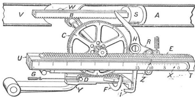
FIG. 15. — COMPTEUR TYPO-MÉTRIQUE
