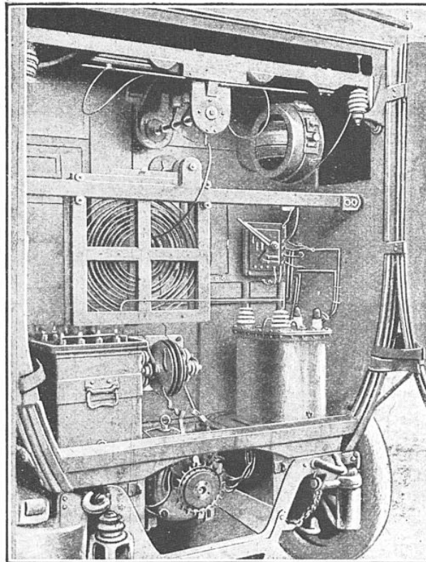
POSTE MOBILE ÉMETTEUR, A ÉTINCELLE
