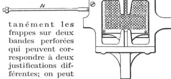
FIG. 22. — LE PORTE-MATRICES ET LES DEUX TIGES QUI EN COMMANDENT LES DÉPLACEMENTS
