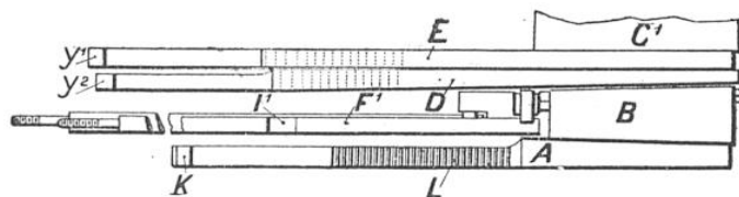
FIG. 26. — POSITIONS RELATIVES DU COIN NORMAL DE RÉGLAGE, DES COINS JUSTIFICATEURS ET DU COIN TOTALISATEUR (VUE EN PLAN).
