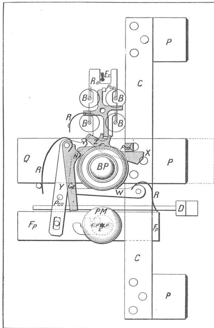
FIG. 19. — SERRURE DE COFFRE-FORT BAUCHE DANS SA POSITION D'OUVERTURE
