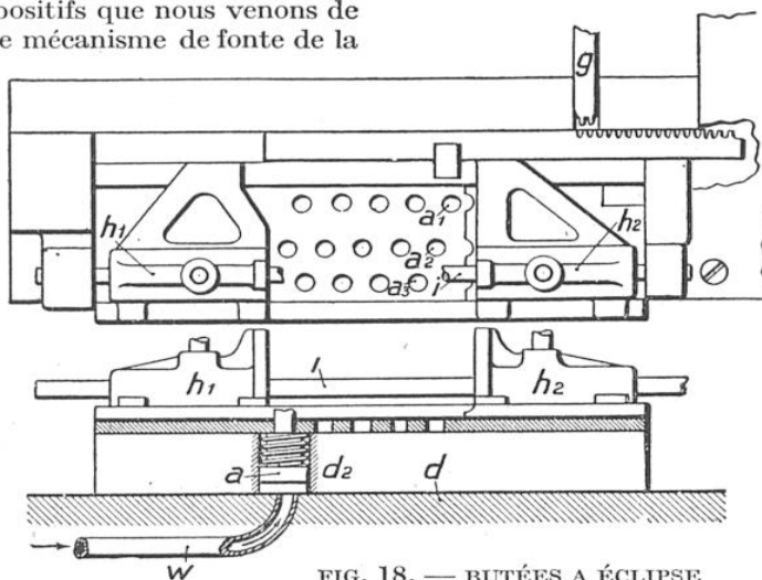
FIG. 18. — BUTÉES A ÉCLIPSE CONTROLANTE LA POSITION DU PORTE-MATRICES
