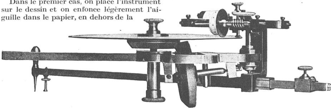
VUE, SOUS UN AUTRE ASPECT, DE LA PARTIE GAUCHE DU PLANIMÈTRE POLAIRE DU TYPE AMSLER, A DISQUE TOURNANT, DONT L'ENSEMBLE EST REPRÉSENTÉ PAR LA FIGURE SUPÉRIEURE. La roulette intégrante est actionnée ici par l'intermédiaire d'un disque entraîné lui-même par un galet conique roulant sur la surface du plan. La sensibilité de l'appareil est grande grâce à l'emploi du disque qui amplifie dans une forte proportion les déplacements du galet conique.
