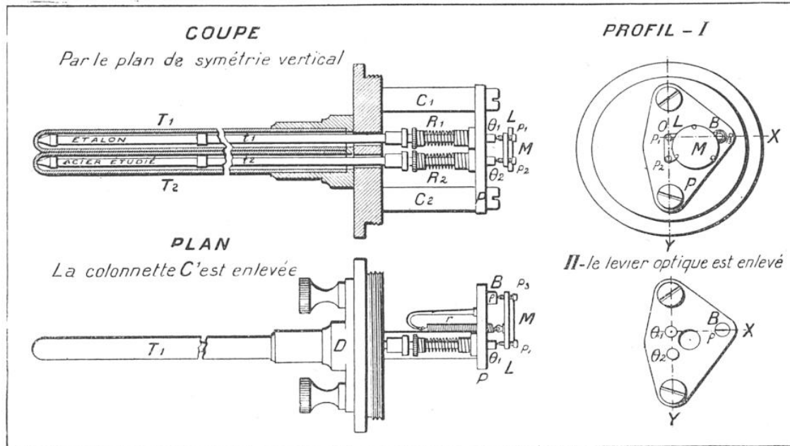
COUPES ET PROFILS DU DILATOMÈTRE ENREGISTREUR CHEVENARD
