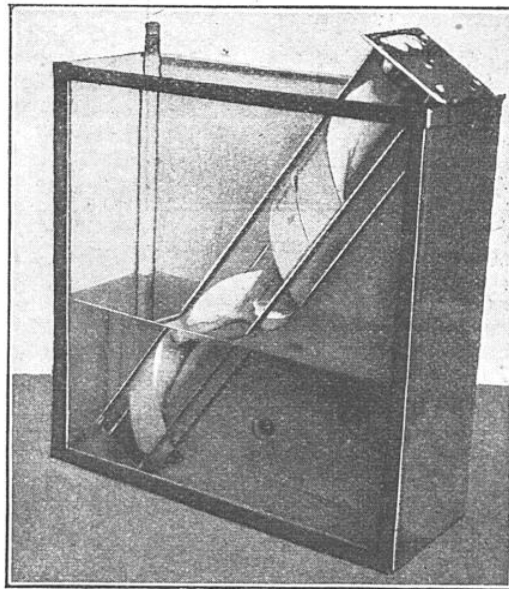
CET INDICATEUR DE NIVEAU EST BASÉ SUR L'ÉQUILIBRE QUE PREND, DANS UN LIQUIDE, UN CORPS ENROULÉ EN HÉLICE AUTOUR D'UN AXE INCLINÉ
