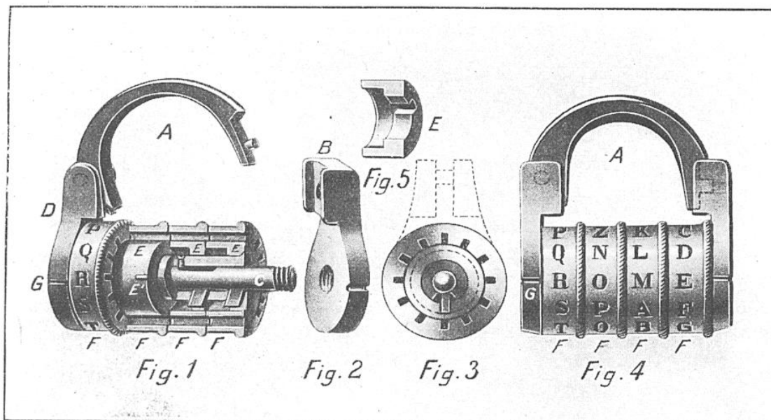
PLANCHE 7. — TYPE COURANT DE CADENAS A COMBINAISONS
