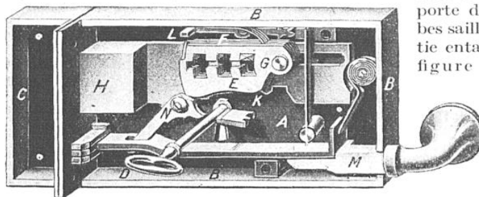
FIG. 2. — SERRURE DE SÛRETÉ FICHET A GARDES MOBILES E , gardes mobiles capables d'osciller autour d'un axe ; F , ressorts-lames appuyant sur les gardes mobiles ; H , pêne ; C , gâche ; A , palâtre ; L , délateur ; M , bouton du bec-de-cane ; N , levier permettant d'actionner le bec-de-cane avec la clef D .
