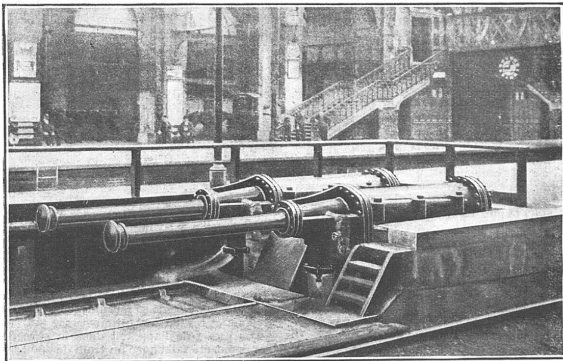
DEUX HEURTOIRS HYDRAULIQUES POUR UNE VOIE TERMINUS, INSTALLÉS DANS LA GARE DE TOURS (COMPAGNIE DU CHEMIN DE FER DE PARIS A ORLÉANS)
