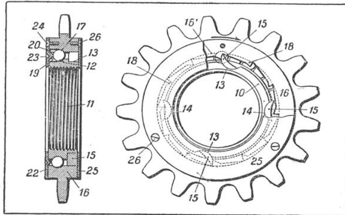
UNE ROUE LIBRE SIMPLE ET ÉTANCHE A LA POUSSIÈRE
