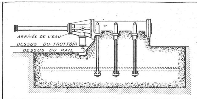
LE HEURTOIR A FREIN HYDRAULIQUE DE LA GARE DE TOURS, VU EN ÉLEVATION ET COUPE PARTIELLE
