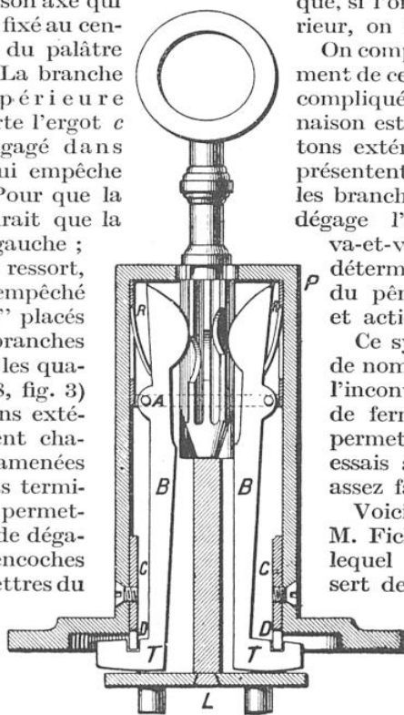
FIG. 15. — PREMIER MODÈLE DE LA SERRURE NOEL-SCAILQUIN
