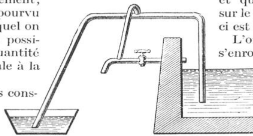
SIPHON S'AMORÇANT AUTOMATIQUEMENT QUAND L'EAU ARRIVE AU NIVEAU DU PETIT TUBE TRAVERSANT LA PAROI
