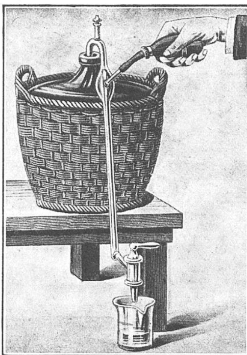
SIPHON PNEUMATIQUE A ROBINET DE P. ROUSSEAU ET A. LELIÈVRE
