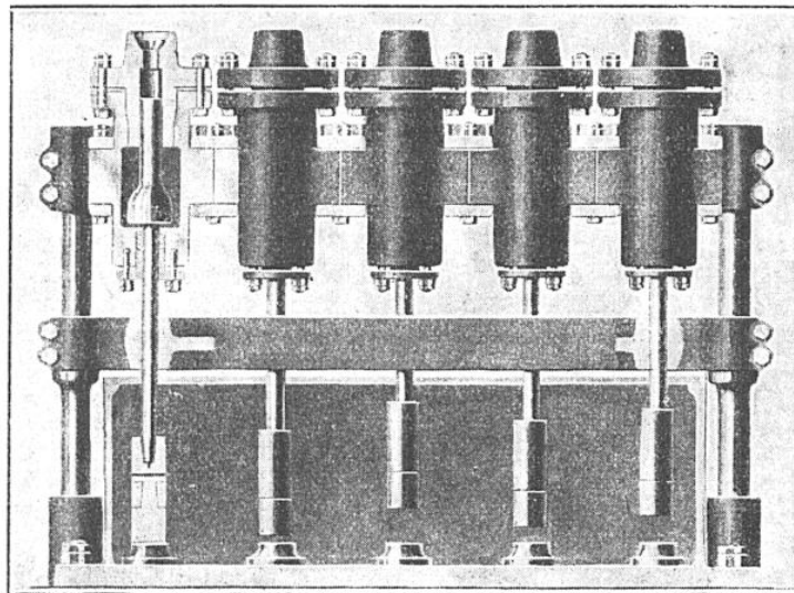
BATTERIE D'ESTAMPEUSES ACTIONNÉES PAR VIBRATIONS
