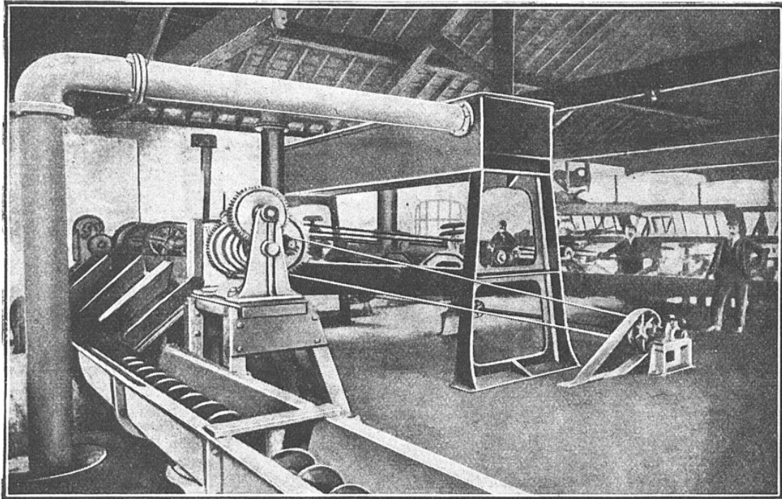
TÊTES DES COULOIRS DE LAVAGE « ELLIOT » VERS LESQUELLES LES PALETTES DES CHAINES FONT REMONTER LES PIERRES ET AUTRES IMPURETÉS
