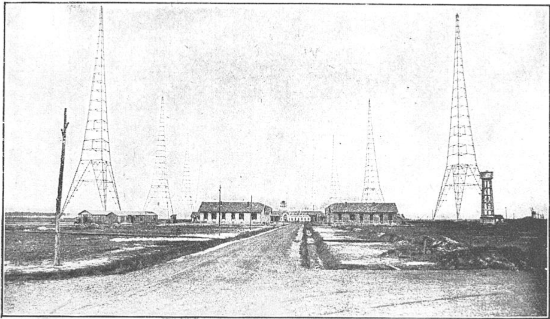
CHAQUE PYLÔNE DU POSTE DE BORDEAUX (EXACTEMENT A CROIX D'HINS) EST UNE VÉRITABLE PETITE TOUR EIFFEL DE 250 MÈTRES DE HAUT. L'ÉMISSION DE CE POSTE GIGANTESQUE EST SUSCEPTIBLE D'ÊTRE ENTENDUE DANS LE MONDE ENTIER
