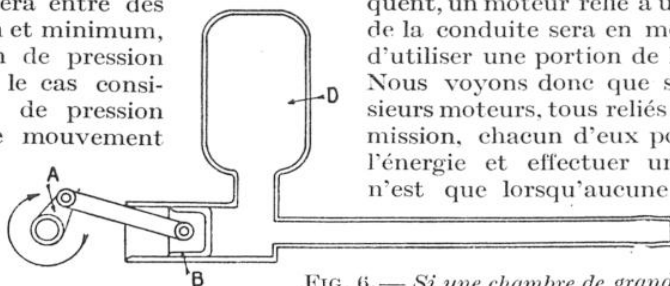
FIG. 6. — Si une chambre de grande capacité, remplie de liquide, est reliée à la conduite dans le voisinage du piston, elle absorbera l'énergie des ondes incidentes et réfléchies lorsque la pression dans la conduite tendra à s'élever; elle restituera cette énergie lorsque la pression tendra à s'abaisser. La pression moyenne dans la chambre et dans la conduite sera la même et ne pourra jamais dépasser la valeur limite pour laquelle le système aura été calculé.
