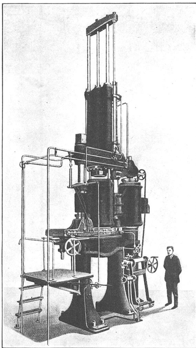
PRESSE HYDRAULIQUE VERTICALE A DEUX CLOCHES Cette machine permet d'obtenir un travail continu, une des cloches, ou cylindres, se remplissant pendant que l'autre débite son produit par la filière inférieure.
