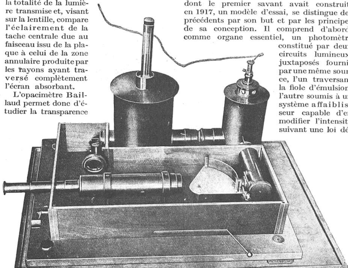
VUE DE L'OPACIMÈTRE VLÈS, DE WATTEVILLE ET LAMBERT, DÉMONTÉ
