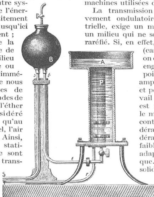
FIG. 1. — DISPOSITIF A L'AIDE DUQUEL WERTHEIM DÉMONTRA, EN 1848-1851, QUE LES TUYAUX REMPLIS D'EAU PEUVENT DONNER DES SONS ET, PAR CONSÉQUENT, TRANSMETTRE DE L'ÉNERGIE PAR VIBRATIONS
