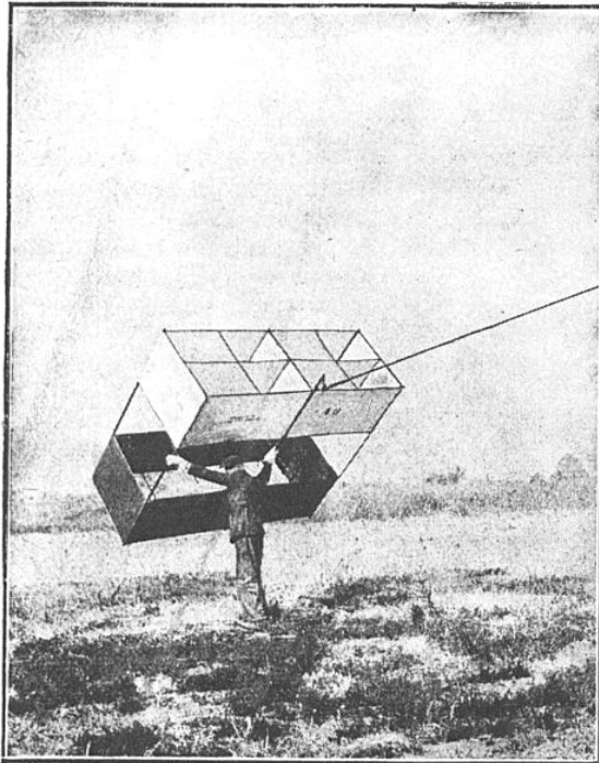
CERF-VOLANT MARVIN SPÉCIALEMENT UTILISÉ AUX ÉTATS-UNIS
