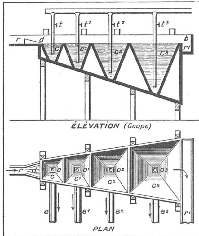
SPITZKASTEN, COUPE EN ÉLEVATION (EN HAUT) ET VUE EN PLAN (AU-DESSOUS)
