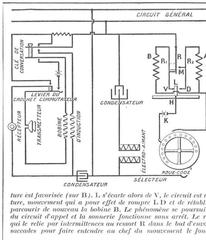
FIG. 5. — SCHÉMA DES COMMUNICATIONS ÉLECTRIQUES D'UN POSTE DE STATION ÉQUIPÉ AVEC UN SÉLECTEUR
