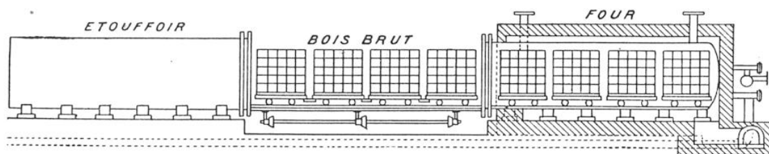
FOUR HORIZONTAL (EN COUPE) AVEC ÉTOUFFOIR ET CHARIOT TRANSBORDEUR
