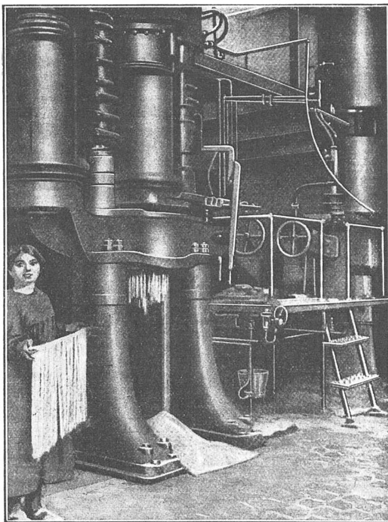
LE MACARONI SE FAIT MÉCANIQUEMENT
