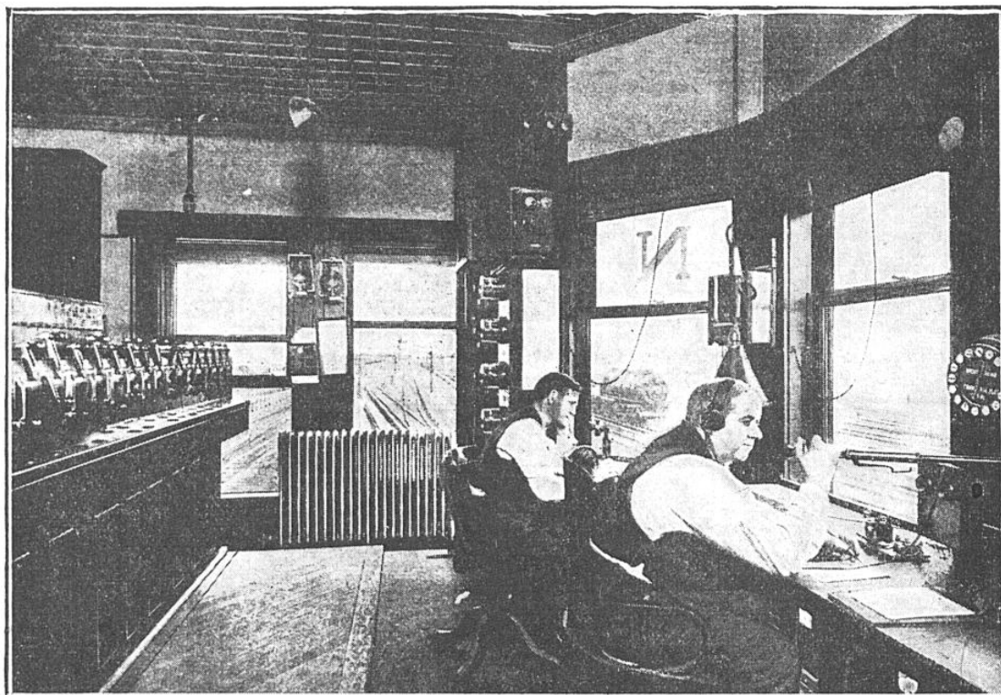
FIG. 11. — LE CHEF DU POSTE D'AIGUILLAGE EST EN RELATIONS CONSTANTES AVEC LE CHEF DU MOUVEMENT DES TRAINS SUR LA LIGNE
