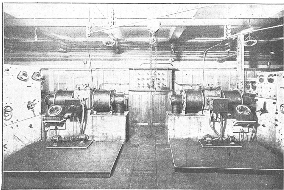
LES DEUX ARCS CHANTANTS DU POSTE DE T. S. F. DE LA TOUR EIFFEL
