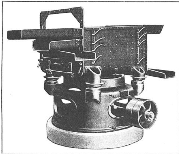
CRIBLE GIRATOIRE, SYSTÈME COXE, CONSTRUIT PAR M. PINETTE
