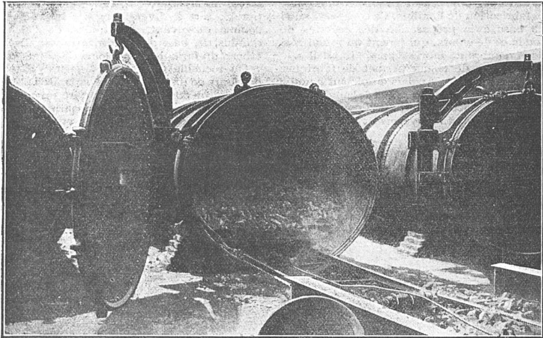
VIDANGE D'UN ÉTOUFFOIR APRÈS LE REFROIDISSEMENT DE SON CONTENU
