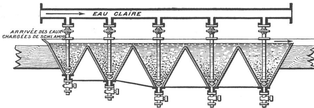
SPITZKASTEN DÉCANTEURS DE « SCHLAMMS » CONSTRUITS PAR LES ATELIERS COPPÉE
