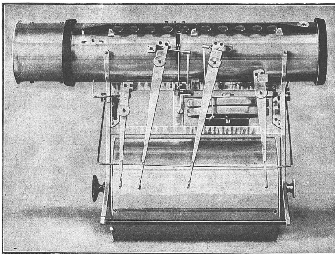
MÉTÉOROGAPHE AMÉRICAIN MARVIN POUR LE SONDAGE DE L'ATMOSPHERE
