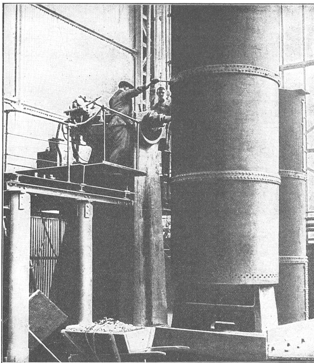
MACHINE HYDRAULIQUE POUR LE RIVETAGE DES ÉLÉMENTS DE CHAUDIÈRES
