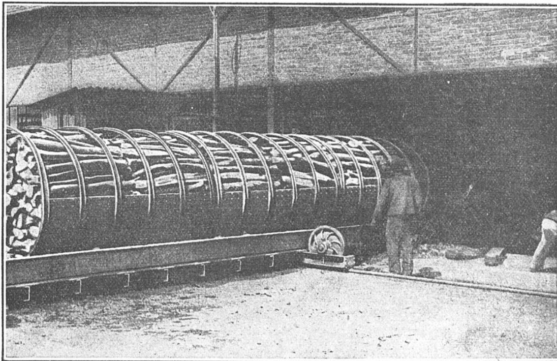
INTRODUCTION DU BOIS DANS UNE CORNUE DE DISTILLATION HORIZONTALE
