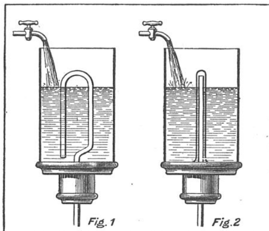
VERRES DE TANTALE SE VIDANT AUTOMATIQUEMENT QUAND LE NIVEAU DE L'EAU ATTEINT LE SOMMET DU SIPHON
