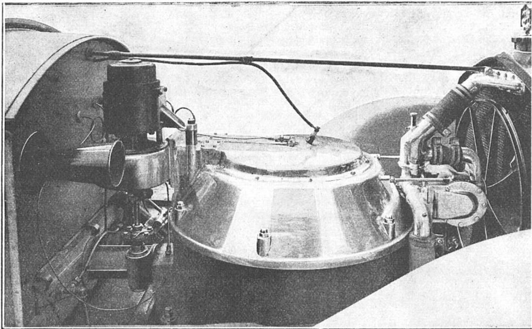
CHAUDIÈRE (RECOUVERTE DE SON ENVELOPPE), RADIATEUR-CONDENSEUR, MOTEUR DES POMPES ET QUELQUES AUTRES ACCESSOIRES DE L'AUTOMOBILE NEWCOMB ET SCOTT
