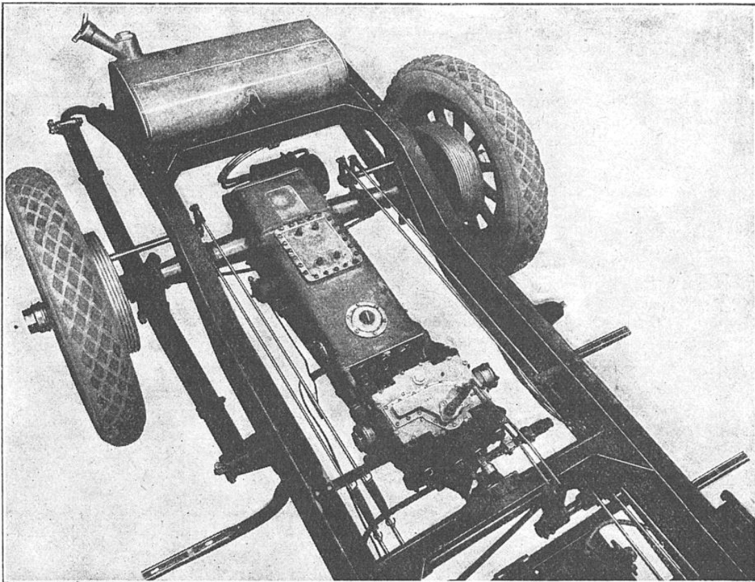
LA MACHINE ET LE PONT ARRIÈRE DE LA NOUVELLE VOITURE A VAPEUR
