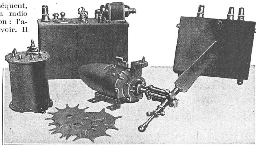
L'ALTERNATEUR DU POSTE PRÉCÉDENT AVEC TOUS SES ACCESSOIRES
