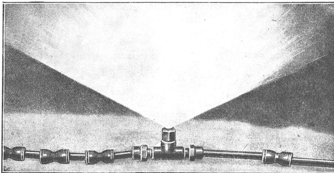
JET D'EAU PULVÉRISÉ POUR ABATTRE LA POUSSIÈRE DANS LES MINES
