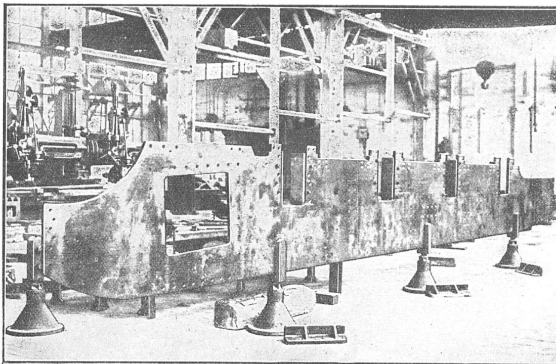
VÉRIFICATION ET DRESSAGE D'UN LONGERON POUR UNE PUISSANTE LOCOMOTIVE
