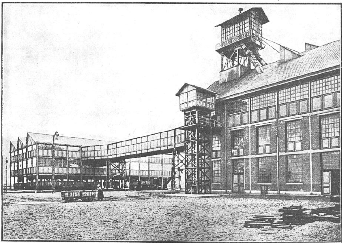
VUE EXTÉRIEURE D'UNE INSTALLATION DE TRIAGE ET DE LAVAGE DE CHARBONS AUX MINES DE LENS (CETTE INSTALLATION A ÉTÉ COMPLÈTEMENT DÉTRUITE PAR LES ALLEMANDS)
