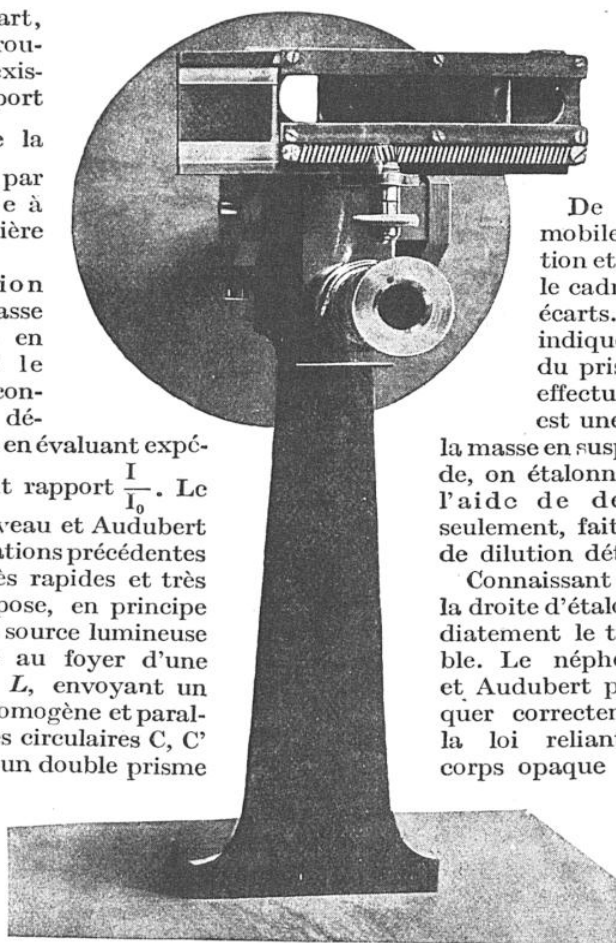
LA LAME OPAQUE DU NÉPHÉLÉMÈTRE
