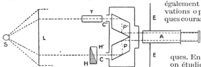
COUPE SCHÉMATIQUE DU NÉPHÉLÉMÈTRE CHÉNEVEAU ET AUDUBERT (1920)
