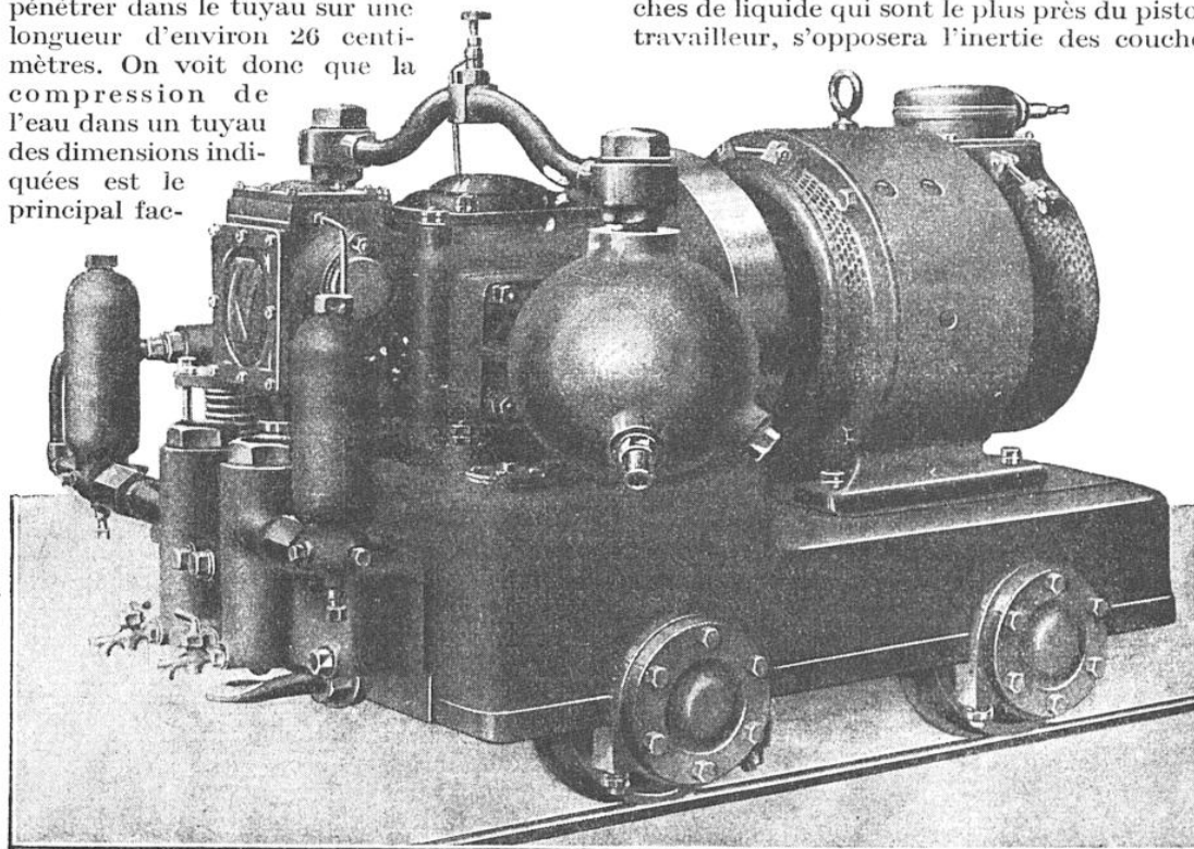
VUE D'ENSEMBLE D'UN GÉNÉRATEUR D'ONDES DE 10 CHEVAUX ET 40 PÉRIODES, ACCOUPPLÉ DIRECTEMENT A UN MOTEUR ÉLECTRIQUE D'ENTRAÎNEMENT ET MONTÉ SUR ROUES
