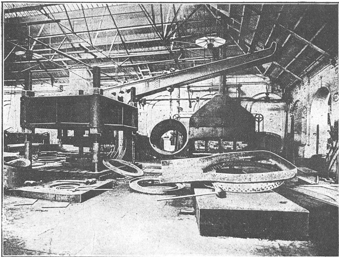
PRESSES HYDRAULIQUES DANS UN ATELIER DE GROSSE CHAUDRONNERIE
