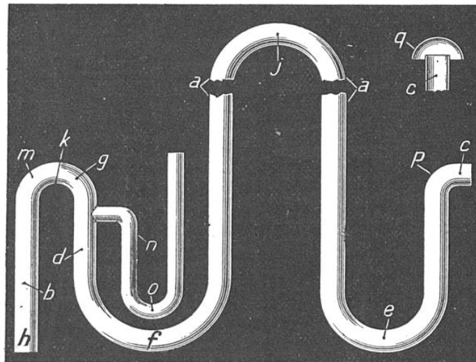
SIPHON DE M. NICHOLSON NE SE DÉSAMORÇANT PAS DANS LE CAS OU L'ORIFICE D'ENTRÉE CESSE D'ÊTRE RECOUVERT PAR LE LIQUIDE
