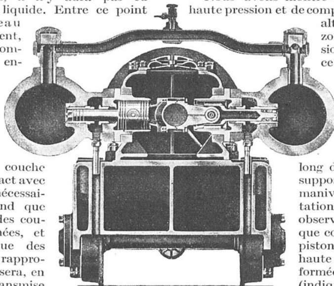
COUPE DU GÉNÉRATEUR, PAR LE TRAVERS DES « CAPACITÉS »
