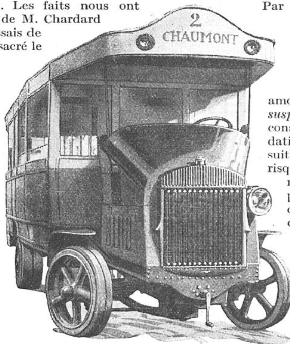
AUTOBUS PARISIEN MUNI DU RADIATEUR A ÉLÉMENTS AMOVIBLES SYSTÈME CHARDARD
