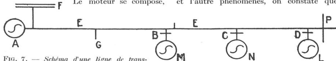
FIG. 7. — Schéma d'une ligne de transmission comportant plusieurs moteurs (M N L) montés en dérivation, c'est-à-dire desservis par des ramifications du conduit principal; chaque moteur est contrôlé par un robinet (B C D) et la conduite peut être fermée complètement en P; A est le générateur et F est une « capacité ».
