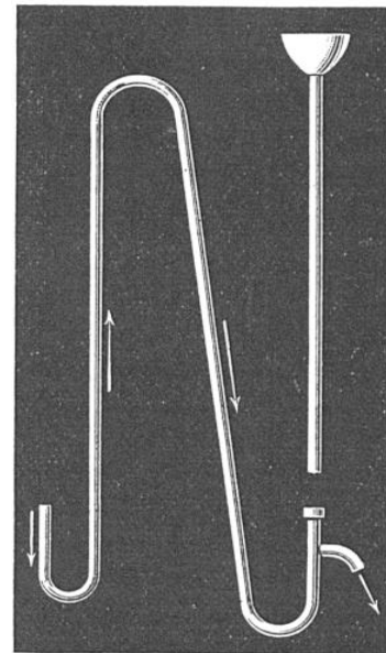
SIPHON DE M. ECHIVARD, RESTANT CONSTAMMENT AMORCÉ
