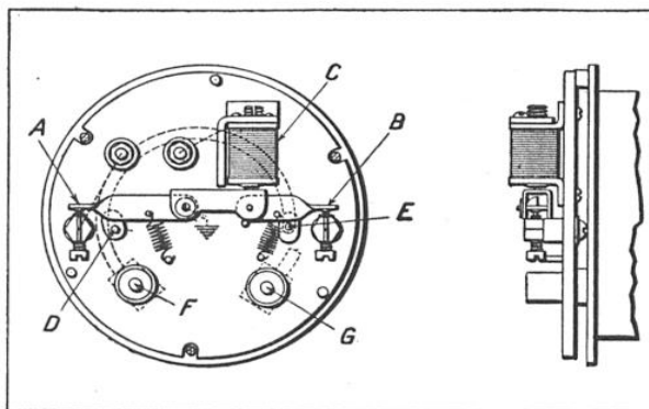
SCHÉMA DES DISPOSITIFS ÉLECTRO-MÉCANIQUES ADAPTÉS A UN MANOMÈTRE BOURDON POUR CONTRÔLER LA PRESSION D'EAU ET DE PÉTROLE A, interrupteur du circuit d'allumage; B, interrupteur du circuit de l'interrupteur électro-magnétique qui contrôle le moteur d'entraînement des pompes; C, électro-relais relié en série avec l'interrupteur électro-magnétique du circuit du moteur; D, butée du tube du manomètre pour le contrôle de la pression du pétrole; E, butée analogue mais contrôlant la pression d'eau; F et G, jonctions aux tuyaux de vapeur et d'eau.
