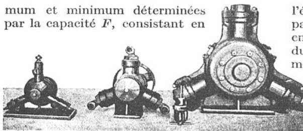
QUELQUES MOTEURS « A VIBRATIONS »
