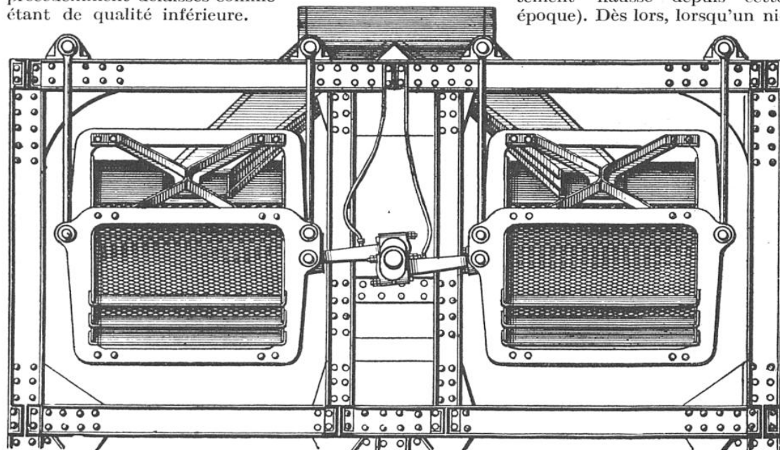
CRIBLE DOUBLE, A SECOUSSES, CONSTRUIT PAR M. EVENCE COPPÉE
