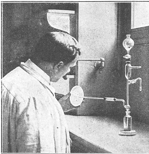
L'ARSENIC PROJETÉ EN TACHES SUR UNE SOUCOUPE On utilisait primitivement l'appareil de Marsh pour produire des taches d'arsenic qui servaient à doser le poison.
