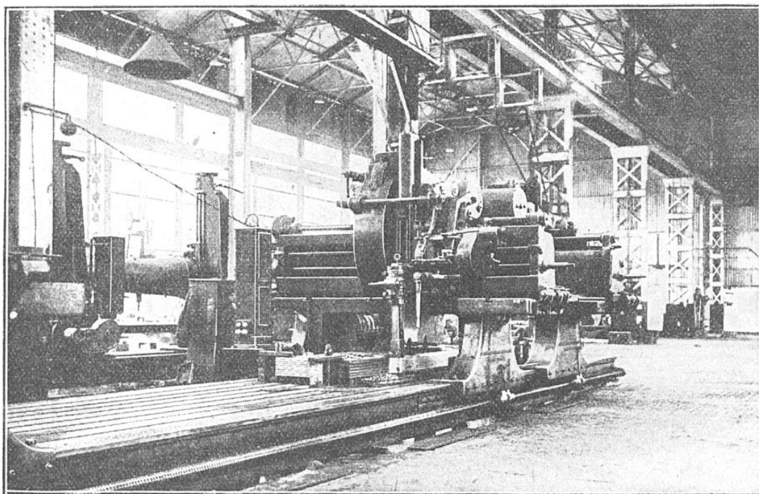
MACHINE-OUTIL POUR LE DÉCOUPAGE DES LONGERONS DES LOCOMOTIVES
