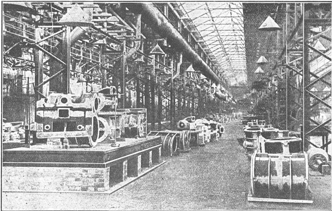
ATELIER SPÉCIAL OU S'EFFECTUE L'USINAGE DES CYLINDRES DE LOCOMOTIVES Au sortir de la fonderie, les cylindres sont alésés et dressés par de nombreuses machines-outils.
