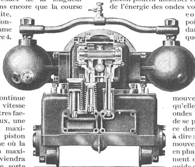
COUPE PAR LE TRAVERS DU CARTER DES ENGRENAGES DE LA POMPE
