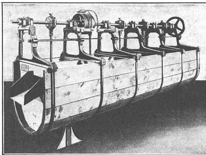
BAC À PISTONS INDUSTRIEL, COMPORTANT CINQ COMPARTIMENTS COMMUNICANTS, DE M. MOREL
