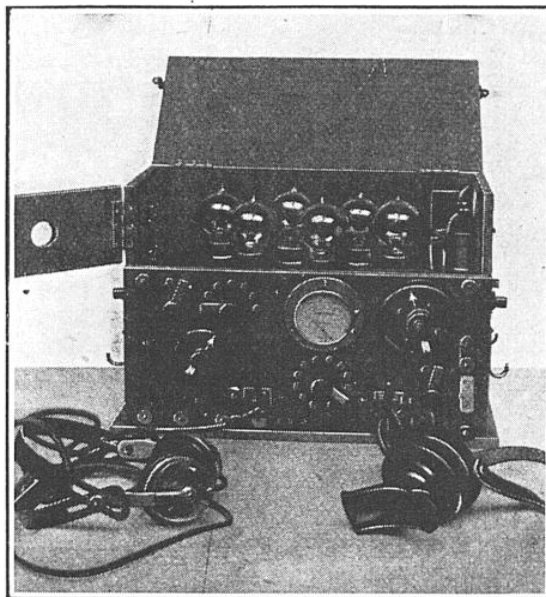
POSTE DE TÉLÉPHONIE SANS FIL POUR AVION AYANT RÉALISÉ QUINZE KILOMÈTRES DE PORTÉE ENTRE APPAREILS (AU PREMIER PLAN LE CASQUE DE RÉCEPTION ET LE MICROPHONE TRANSMETTEUR)
