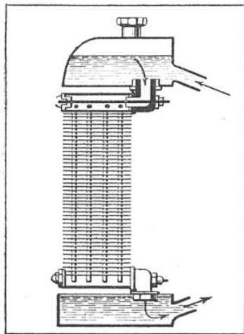
FIG. 2. — CIRCULATION DE L'EAU DANS L'ÉLÉMENT L'eau circule de haut en bas comme dans un radiateur ordinaire.
