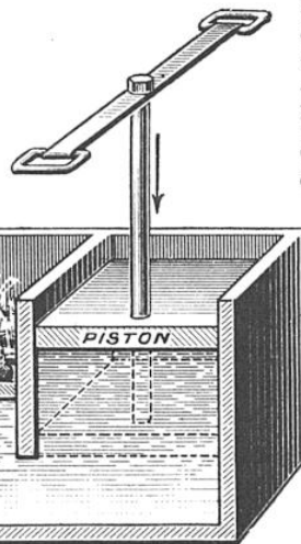
BAC LAVEUR A PISTON, TRÈS SIMPLE, FONCTIONNANT A LA MAIN
