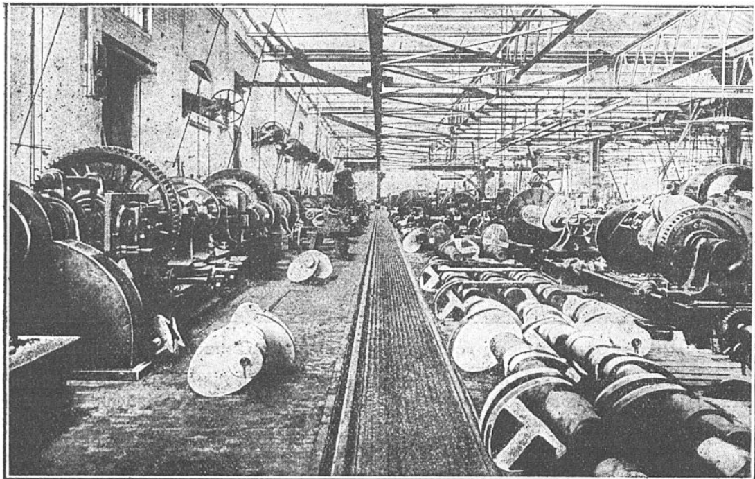
CE HALL EST DESTINÉ A L'USINAGE DES ESSIEUX COUDÉS DE LOCOMOTIVES Les corps et les manivelles des essieux doivent être tournés et dressés avec la plus grande précision.
