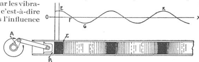
FIG. 3. — Dans une colonne liquide, le va-et-vient d'un piston engendre une succession de zones de compression (en noir) séparées par des zones plus longues de basse pression (en plus clair). Chaque zone de compression se propage en avant du piston le long de la colonne, de sorte que, en tout point de cette dernière, la pression passe par une série de variations qui peuvent être représentées par la courbe sinusoïdale O X et assimilées à une série d'ondes.
