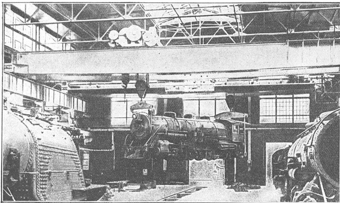
PONT TRANSBORDEUR DE 125 TONNES DANS UN « MONTAGE » DE LOCOMOTIVES
