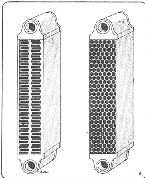
FIG. 1. - LES ÉLÉMENTS DU BLOC REFROIDISSEUR SONT FORMÉS DE TUBES À AILETTES, LAMES ONDULÉES, NIDS D'ABEILLES, ETC.
