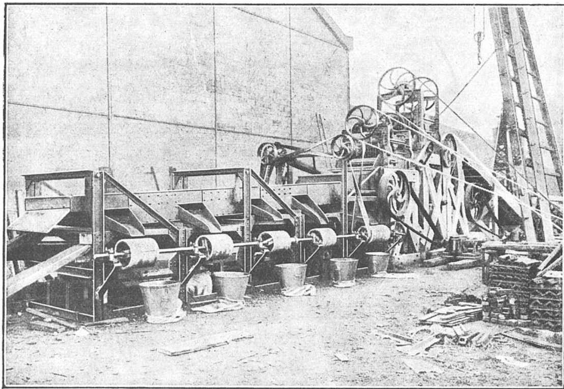
TRIEUR ET CLASSEUR DE M. ALRICQ, POUR LE CHARBON OU L'ANTHRACITE
