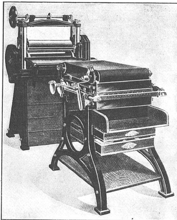
LAMINOIR A CYLINDRES LISSES POUR NOUILLES
