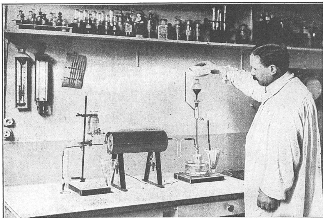
L'APPAREIL DE MARSH QUI DÉCÈLE LES PLUS PETITES TRACES D'ARSENIC
