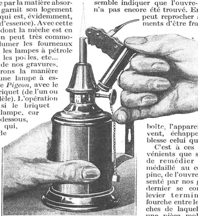
ALLUMAGE D'UNE LAMPE PIGEON AU MOYEN DU BRIQUET
