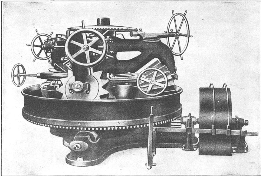
PÉTRIN A ROULEAUX CANNELÉS RÉGLABLES : IL EST TOUJOURS FACILE DE RÉGLER LES ROULEAUX MÊME QUAND LA MACHINE EST EN MARCHÉ ET CHARGÉE
