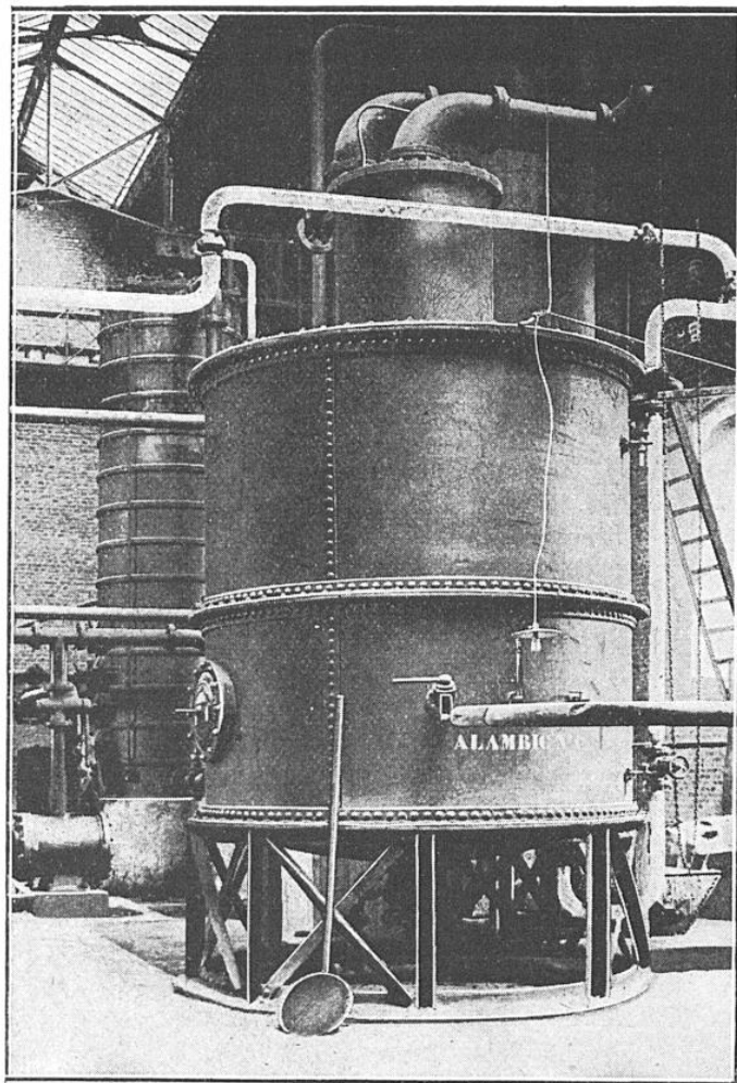
APPAREIL A BARBOTAGE POUR LE DÉGOUTRONNAGE DES DIVERS GAZ PROVENANT DE LA DISTILLATION DU BOIS Comme la plupart des réservoirs des usines établies pour le traitement du liquide résultant de la condensation des vapeurs sortant des cornues, ou pyroligneux, cet alambic est en cuivre épais. On se rend compte du prix de revient élevé d'une semblable installation.
