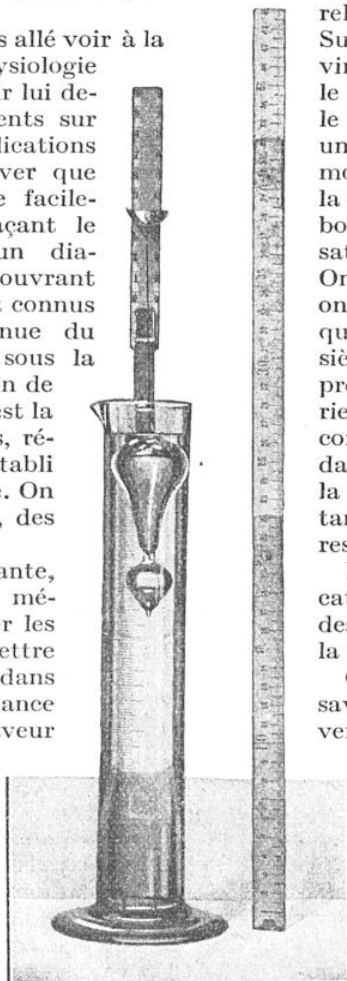
FIGURE 2. — PÈSE-VAPEUR Aréomètre d'une grande sensibilité, dont la tige d'acier nickelé se déplace dans l'alcool le long d'une règle divisée en millimètres.
