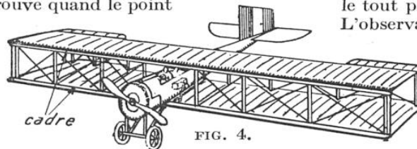
AVION MUNI D'UN CADRE RADIOGONIOMÉTRIQUE Les deux extrémités du cadre sont fermées sur un appareil récepteur disposé dans la carlingue.
