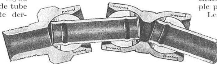
COUPE TRANSVERSALE DU TUYAU FLEXIBLE
