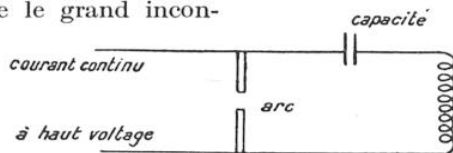
FIG. 7. — L'ARC CHANTANT DE DUDDEL. Le courant continu qui alimente l'arc donne naissance, dans le circuit self-capacité, à un courant alternatif dont la fréquence est liée aux constantes électriques du système.
