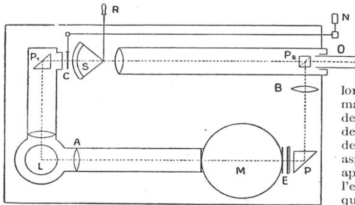
PLAN SCHÉMATIQUE DE L'OPACIMÈTRE VLÈS, DE WATTEVILLE ET LAMBERT (1919)
