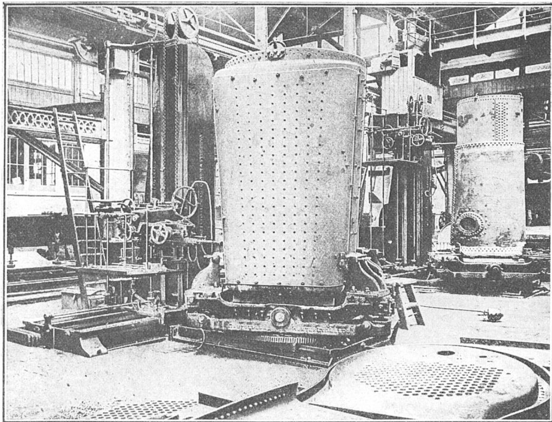
MACHINES A PERCER SPÉCIALES POUR FOYERS ET CORPS DE CHAUDIÈRES
