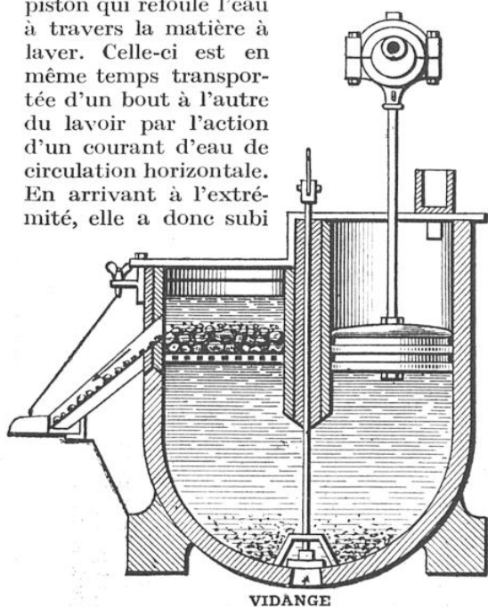
COUPE DE L'UN DES COMPARTIMENTS DU BAC À PISTONS SYSTÈME MOREL
