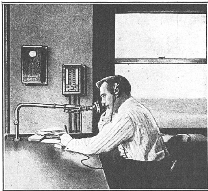
FIG. 13. — POSTE TÉLÉPHONIQUE DE STATION On voit, à gauche, la boîte de sonnerie contenant le sélecteur d'appel. A droite de cette boîte se trouve au petit tableau à jacks et fiches permettant les essais de la ligne et les combinaisons pour rétablir le circuit en cas de dérangement, en utilisant des fils voisins.
