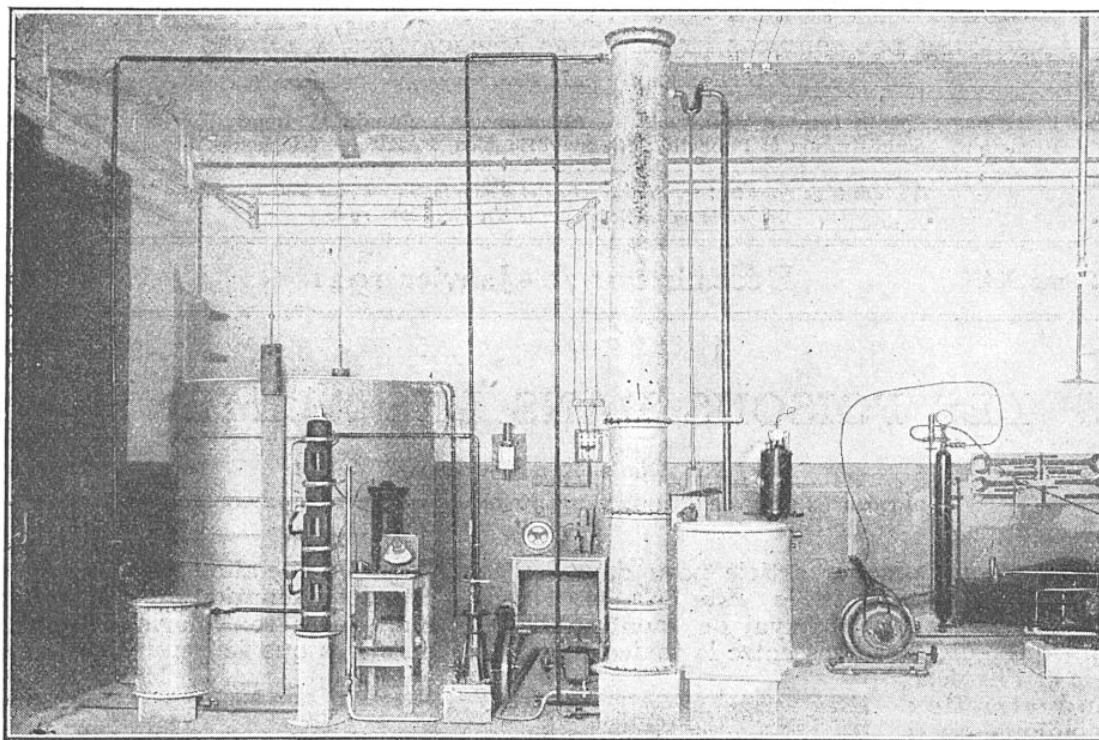
LA STÉRILISATION DE L'EAU PAR L'OZONE AU LABORATOIRE DE M. D'ARSONVAL
