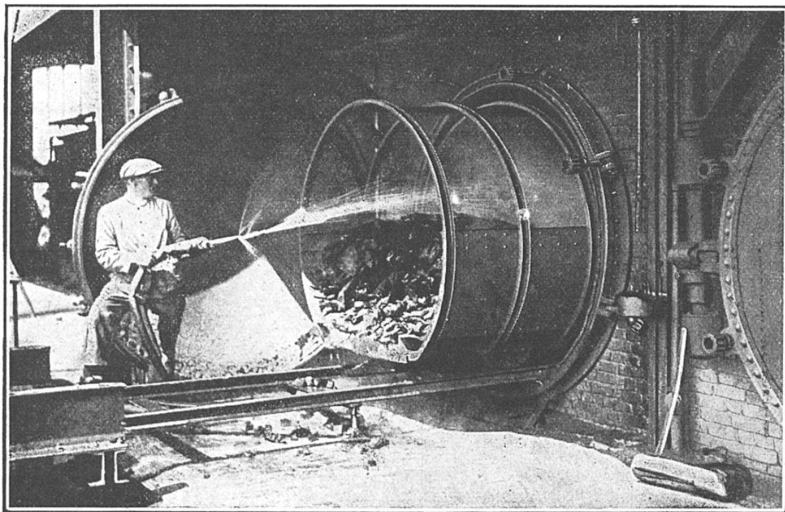
SORTIE DU CHARBON DE LA CORNUE APRÈS LA DISTILLATION DU BOIS
