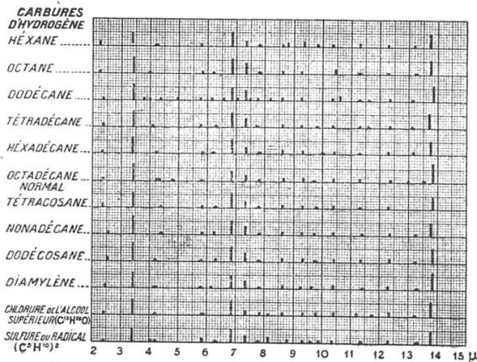
FIG. 5. — SPECTRES INFRA-ROUGES, TOUT À FAIT CONCORDANTS, DES PRODUITS DE LA DISTILLATION DU PÉTROLE. Ces produits ont des odeurs et des saveurs presque identiques.
