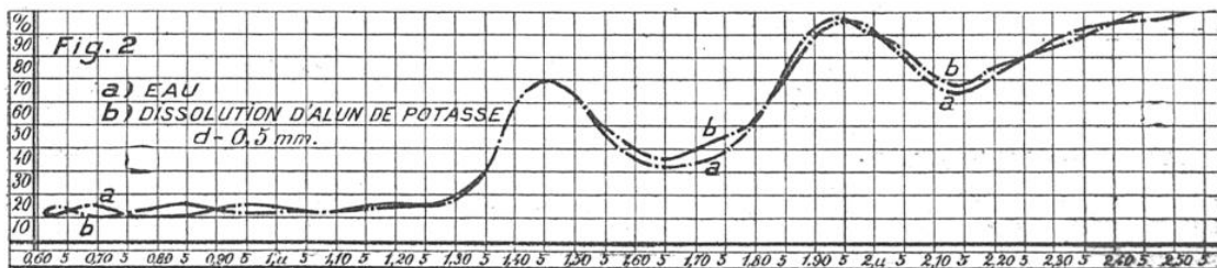
FIG. 6. — SPECTRES D'ABSORPTION DE L'EAU DISTILLÉE ET DE L'ALUN DE POTASSE. L'alun de potasse possède une saveur qui ne diffère de celle de l'eau distillée que par son caractère styptique , qui est une sensation tactile.
