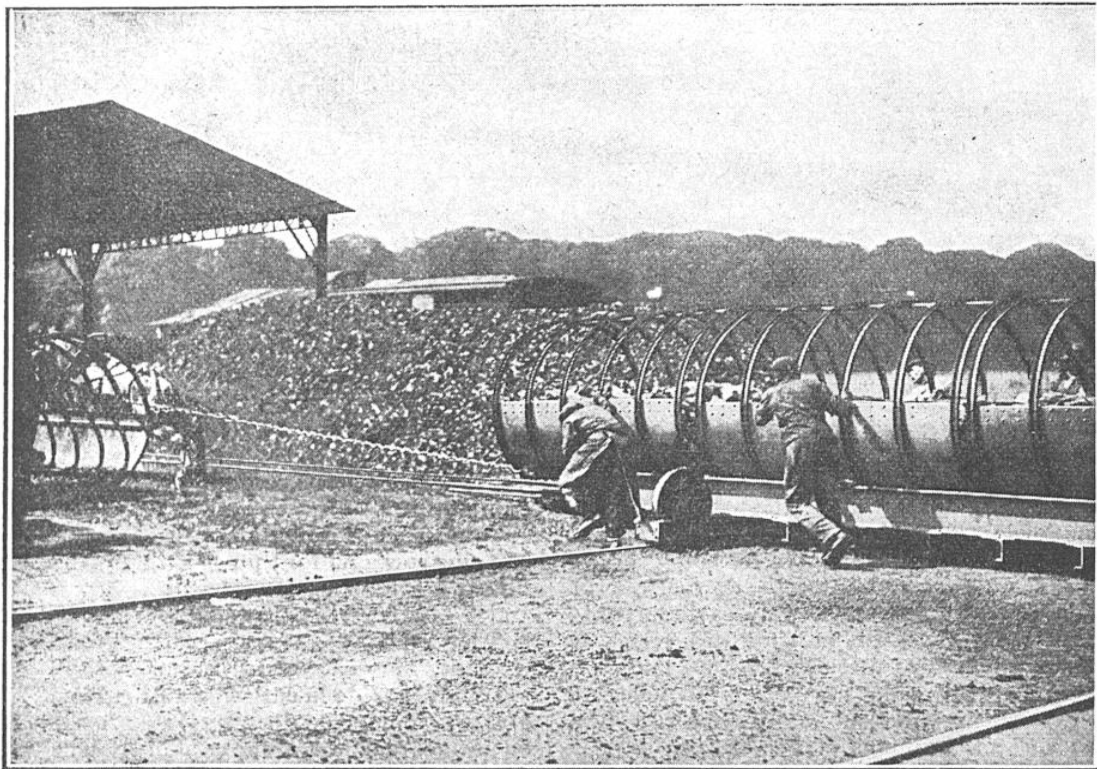
MISE EN TAS DU CHARBON DE BOIS ÉTEINT A SA SORTIE DE L'ÉTOUFFOIR
