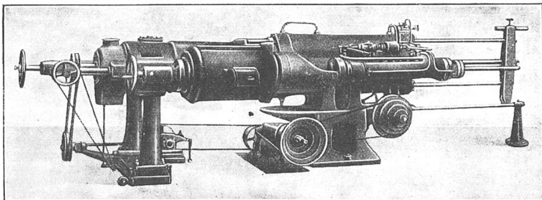
PRESSE HORIZONTALE A DEUX CLOCHES POUR LA FABRICATION DES PÂTES COUPÉES
