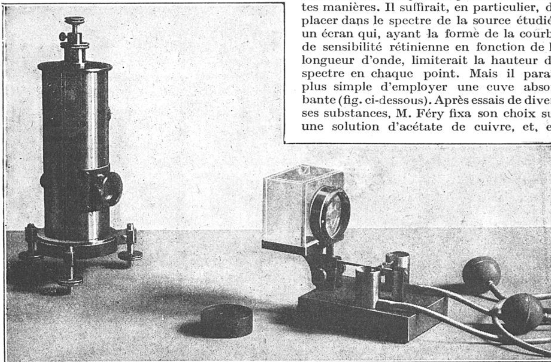
LE PHOTOMÈTRE FÉRY A LECTURE DIRECTE ET LA CUVE ABSORBANTE RENFERMANT UNE SOLUTION D'ACÉTATE DE CUIVRE
