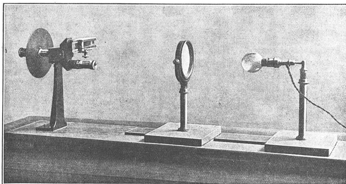
LE NÉPHÉLÉMÈTRE CHÉNEVEAU ET AUDUBERT MONTÉ POUR UNE EXPÉRIENCE A gauche, l'appareil opacimétrique ; au milieu, une lentille ; à droite, la source lumineuse.
