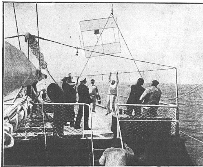
CERF-VOLANT LANCÉ A BORD DE LA « PRINCESSE-ALICE » C'est un appareil cellulaire Hargrave, aux montants duquel on a fixé la boîte qui renferme les instruments.
