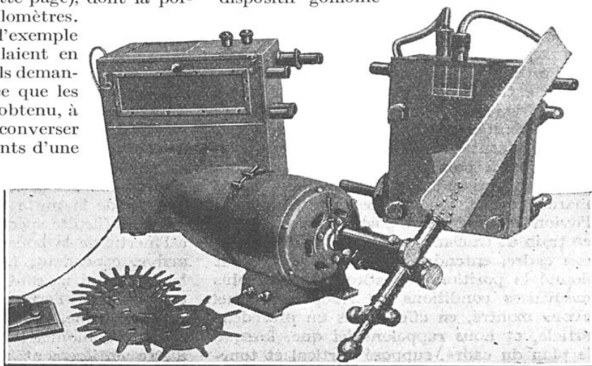
ALTERNATEUR DE 500 WATTS, AVEC SES ACCESSOIRES, POUR AÉRONEFS
