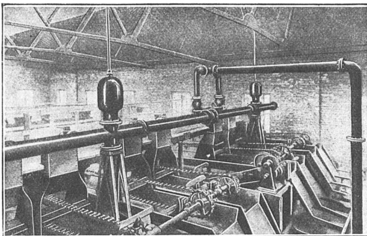
PARTIE INFÉRIEURE DES COULOIRS DE LAVAGE PAR OU SE DÉVERSE LE CHARBON LAVÉ
