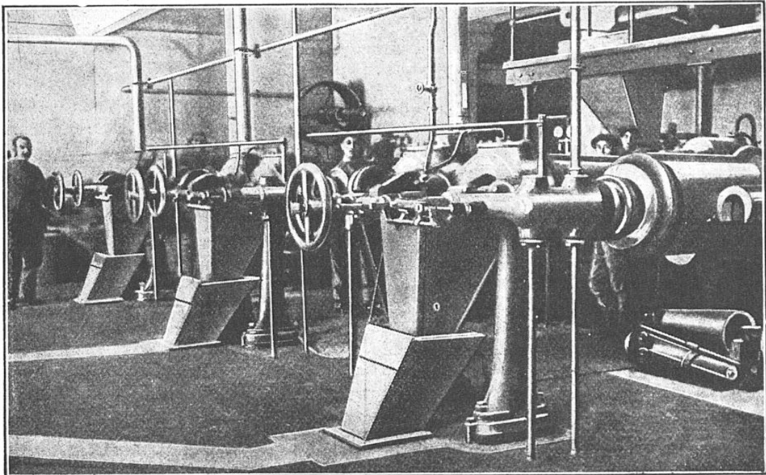
BATTERIE DE PRESSES HORIZONTALES POUR LA FABRICATION DES PÂTES COUPÉES
