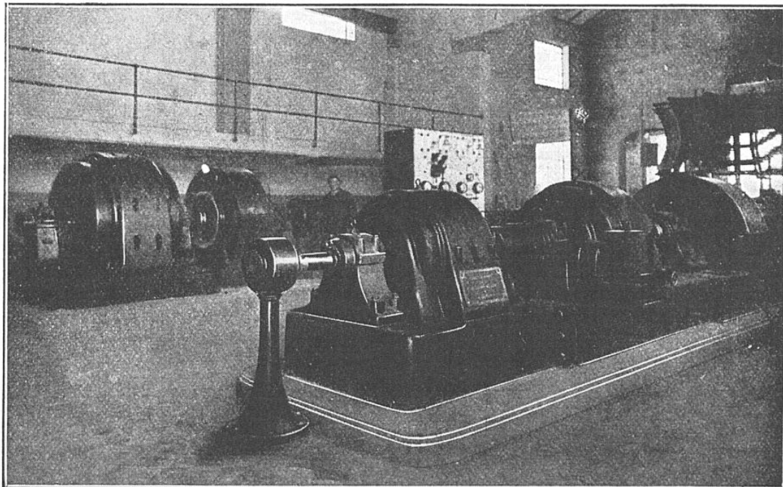
AU PREMIER PLAN, L'ALTERNATEUR A HAUTE FRÉQUENCE DU POSTE DE LYON ; AU DEUXIÈME PLAN LA GÉNÉRATRICE ALIMENTANT LE MOTEUR QUI ENTRAÎNE L'ALTERNATEUR
