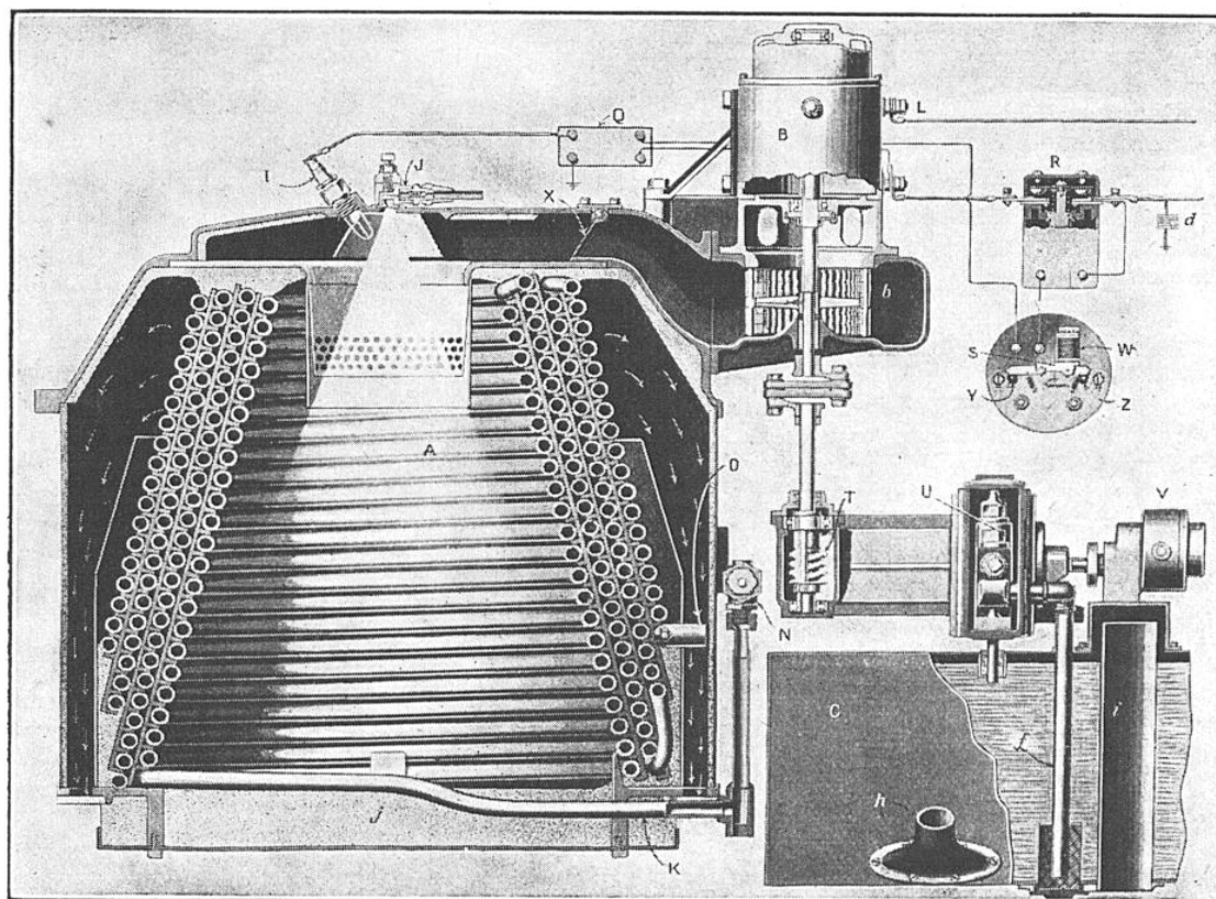
SCHÉMA DE L'APPAREIL ÉVAPORATOIRE ET DE SES DISPOSITIFS DE CONTRÔLE
