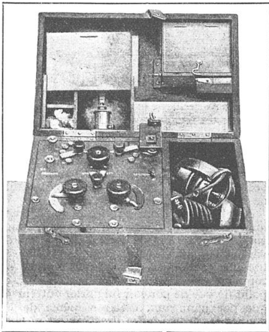
BOITE DE RÉCEPTION UTILISÉE PAR LES GROUPES D'ARTILLERIE ET LES ÉTATS-MAJORS POUR RECEVOIR LES MESSAGES DES AVIONS
