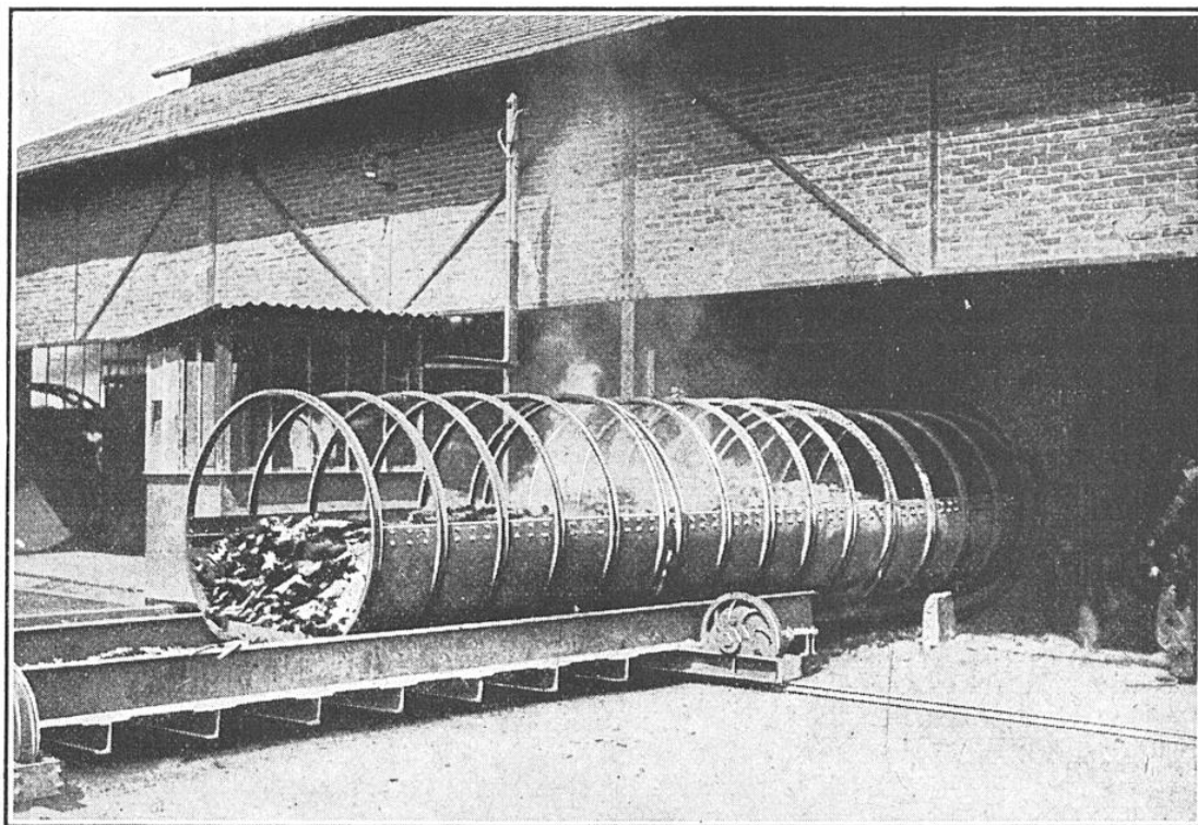
MANŒUVRE D'INTRODUCTION DU CHARBON DE BOIS DANS UN ÉTOUFFOIR
