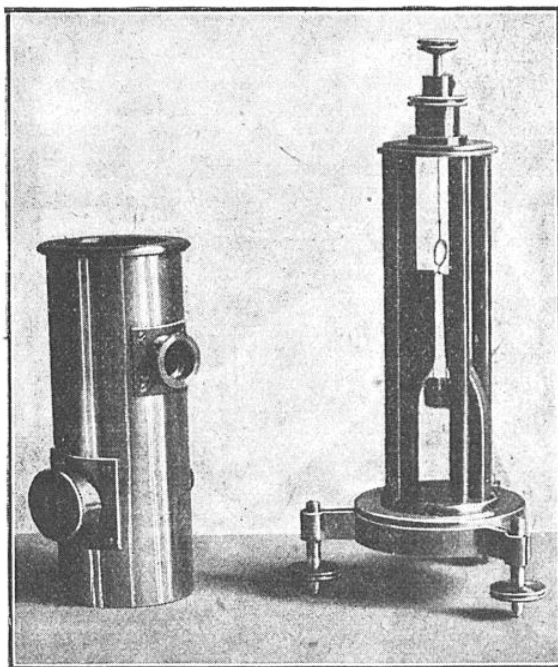
LE PHOTOMÈTRE FÉRY DÉMONTÉ
