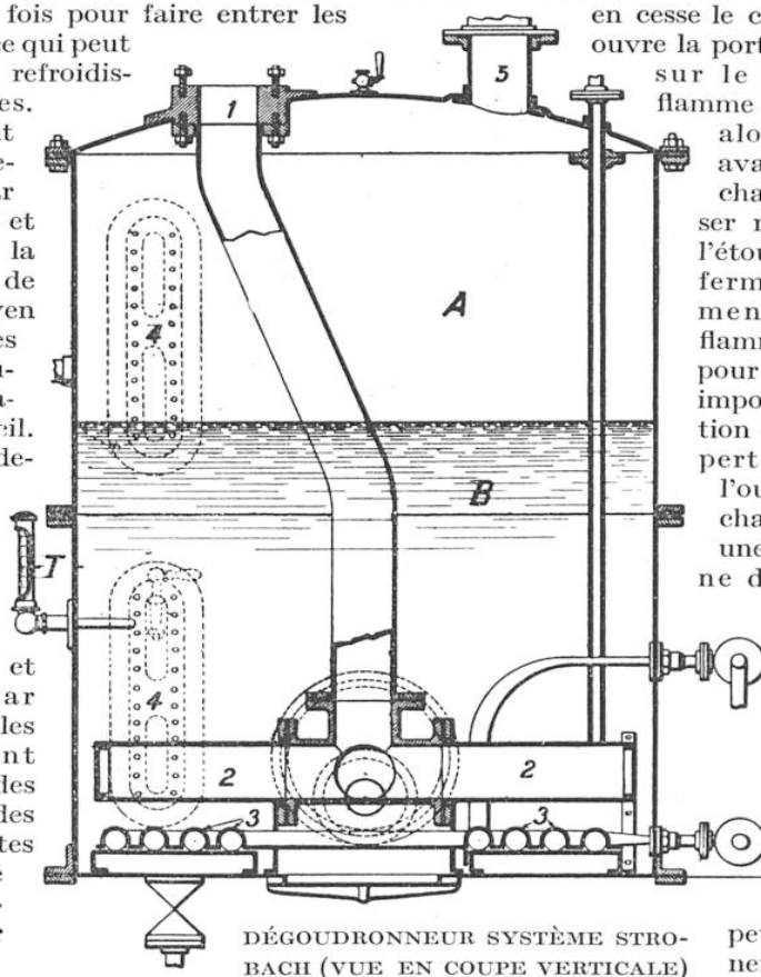
Les vapeurs et les gaz venant des cornues de distillation pénètrent par un tube 1 dans un cylindre en cuivre A B et traversent une couche de goudron d'un mètre d'épaisseur. Les gaz sont divisés dans le liquide par une plaque perforée ou répartis par des tubes perforés 2 montés radialement. On suit le fonctionnement au moyen de glaces 4.
