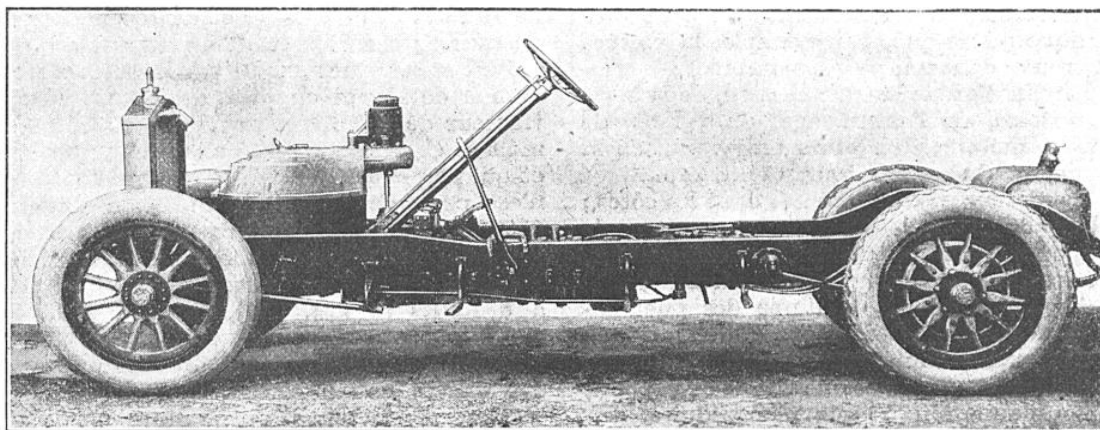
ENSEMBLE DU CHASSIS DE LA NOUVELLE VOITURE AMÉRICAINE A VAPEUR 1
