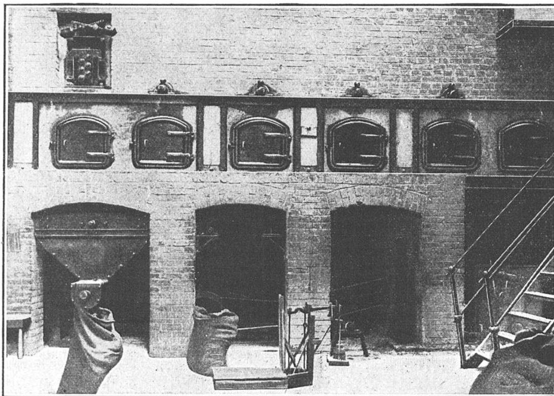
SÉCHOIR HUILLARD POUR LE SÉCHAGE DE L'ACÉTATE DE CHAUX
