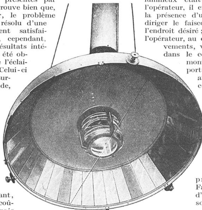
L'OPTIQUE A ÉCHELONS ET LES MIROIRS PLANS
