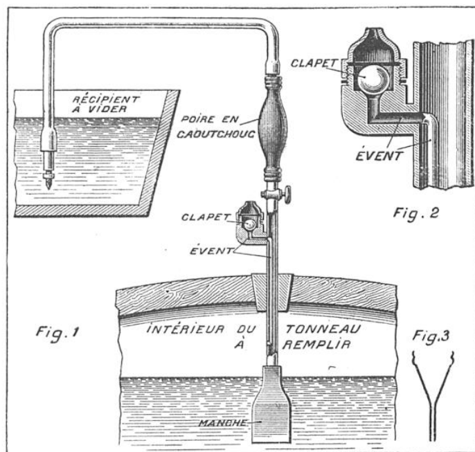
SYSTÈME DE M. KEHRIG POUR ARRÊTER AUTOMATIQUEMENT L'ÉCOULEMENT QUAND LE LIQUIDE SIPHONNÉ ARRIVE A UN NIVEAU DONNÉ
