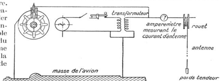
FIG. 2. — POSTE ÉMETTEUR D'AVION POUR RÉGLAGES DU 75 Il se compose essentiellement d'un alternateur mû par une hélice que le mouvement même de l'avion met en rotation, d'un transformateur et d'un éclateur tournant entraîné par l'arbre de l'alternateur. Une étincelle jaillit chaque fois qu'une dent de l'éclateur passe en face d'une l'électrode fixe reliée au secondaire du transformateur.
