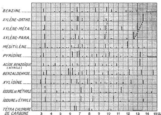
FIG. 8. — SPECTRES D'EXTINCTION DE LA BENZINE ET DE SES PRINCIPAUX DÉRIVÉS
