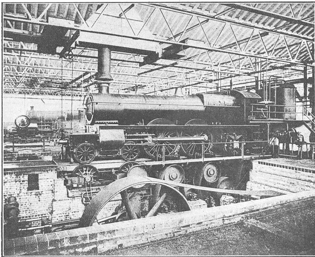
DISPOSITIF POUR L'ESSAI « A FROID » DES LOCOMOTIVES NEUVES OU RÉPARÉES
