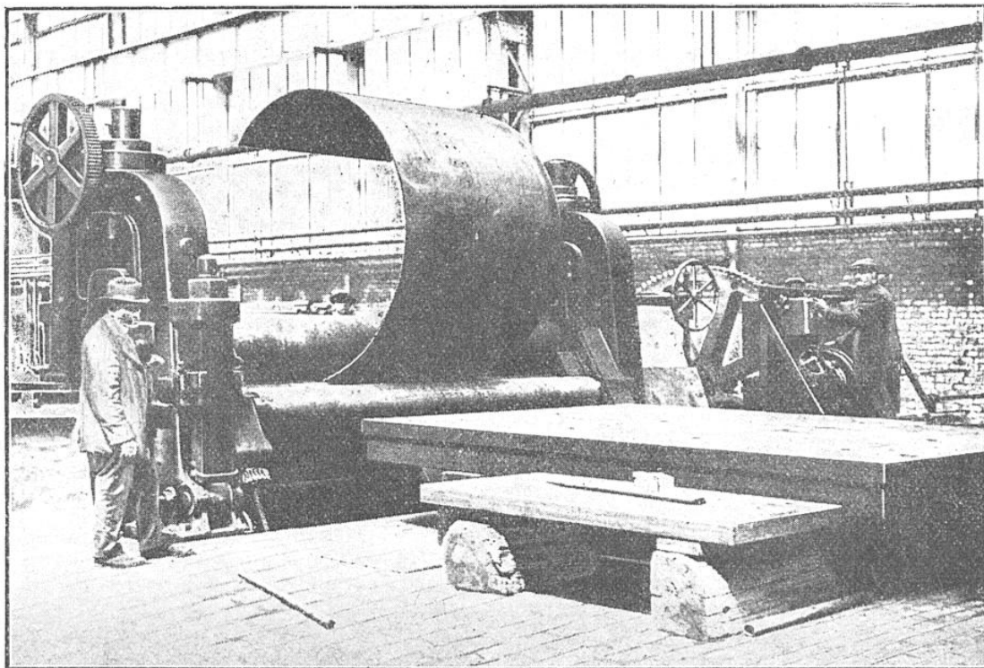
LAMINOIR A FROID POUR ENROULER LES TOLES DE CHAUDIÈRES
