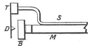
FIG. 8. — VUE EN COUPE DES ORGANES DE COMMANDE DE LA CLÉ DE SÉLECTION
