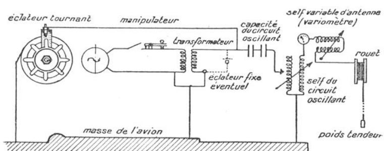
FIG. 3. — POSTE POUR RÉGLAGES DE L'ARTILLERIE LOURDE Pour obtenir des longueurs d'onde plus grandes et une meilleure sélection à la réception, le montage adopté est du type indirect.
