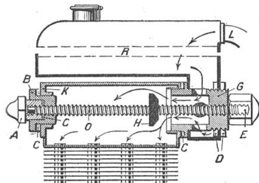
FIG. 3. — SCHÉMA DE MONTAGE R , réservoir ; K , boîte supérieure ; A , contre-écrou ; B , écrou ; C , joints ; D , rondelles ; O , tige filetée ; H , clapet d'arrêt ; G , raccord de fixation ; E , écrou borgne.
