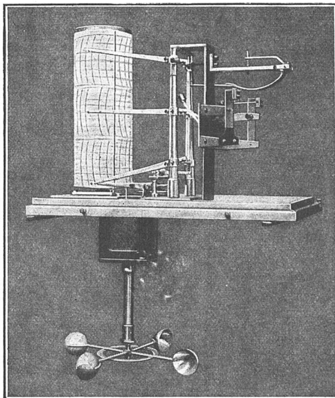
BAROTHERMOHYGROANÉMOMÈTRE RICHARD
