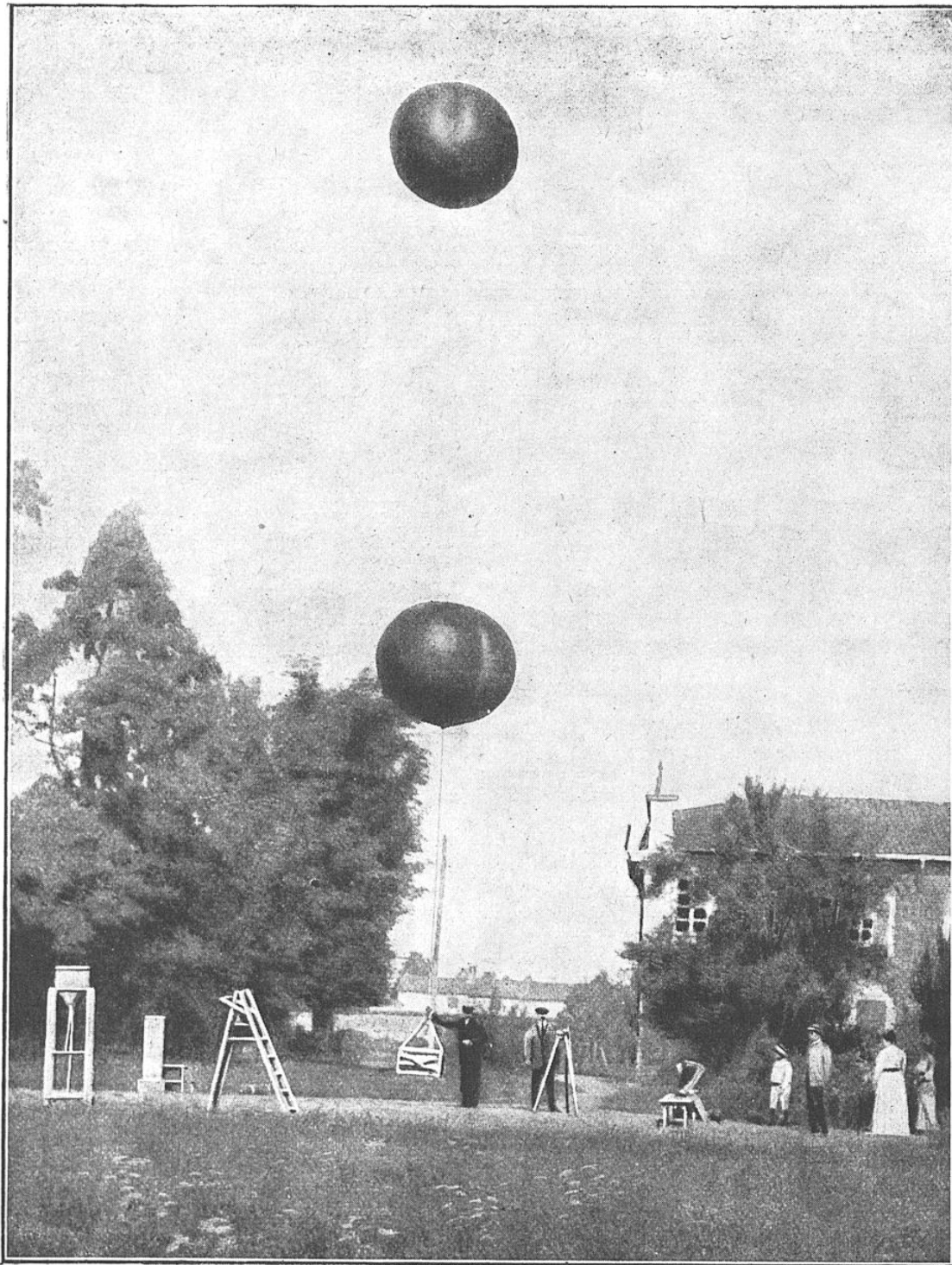
DÉPART DE DEUX BALLONS-SONDES ACCOUPLES A L'OBSERVATOIRE GÉOPHYSIQUE DE PAVIE Le ballon de tête éclate toujours le premier; le ballon inférieur, incapable à lui seul de maintenir les appareils enregistreurs en l'air est cependant suffisant pour ralentir dans de bonnes conditions leur vitesse de chute. Les instruments, relativement fragiles, sont ainsi protégés d'une prise de contact trop violente avec le sol, et le ballon sert encore de repère pour les retrouver.
