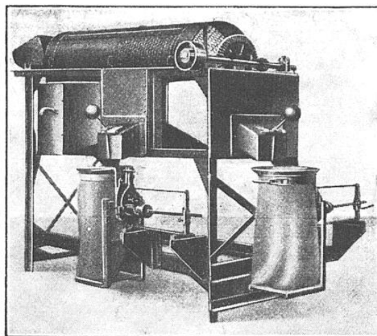
TROMMEL AVEC ENSACHEURS-PESEURS FONCTIONNANT AUTOMATIQUEMENT
