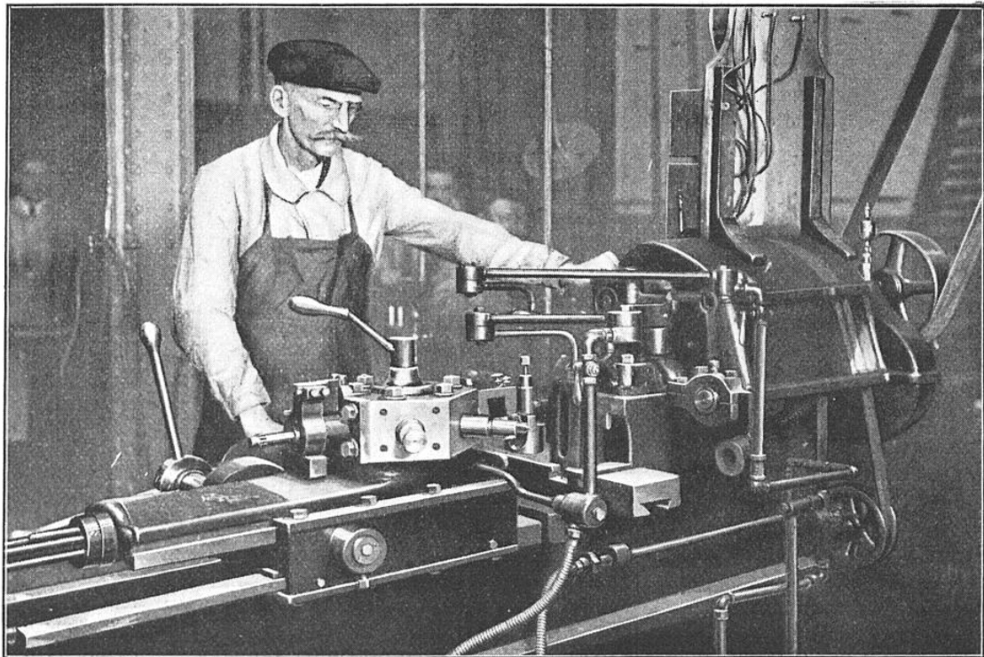
TOUR-REVOLVER A DÉCOLLETER, MONTAGE SEMI-AUTOMATIQUE, POUR L'USINAGE DES PIÈCES PRISES SUR BARRE QUI SERVENT A LA CONFECTION DES AXES D'UNE JUMELLE
