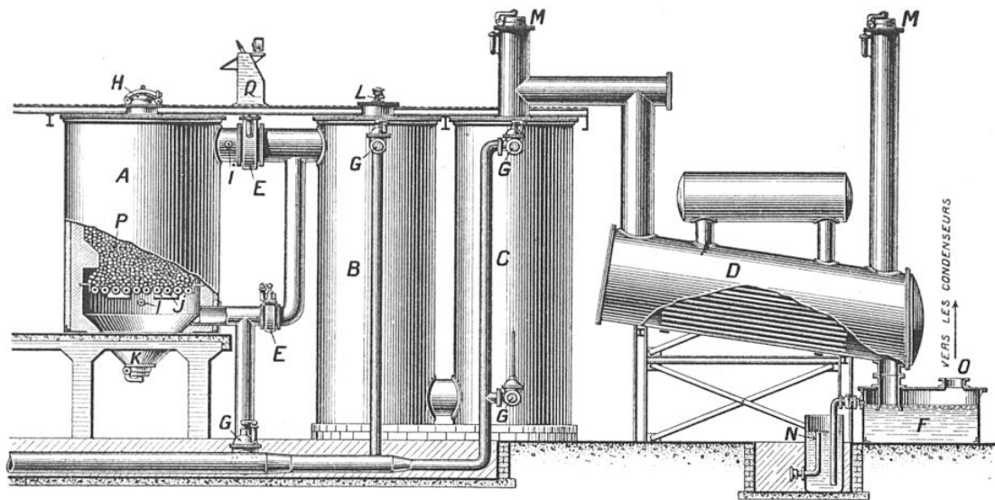
VUE EN ÉLEVATION ET COUPES PARTIELLES D'UNE INSTALLATION DE GAZ A L'EAU DE GRANDE PUISSANCE (TYPE ADOPTÉ PAR LA SOCIÉTÉ DU GAZ DE PARIS)
