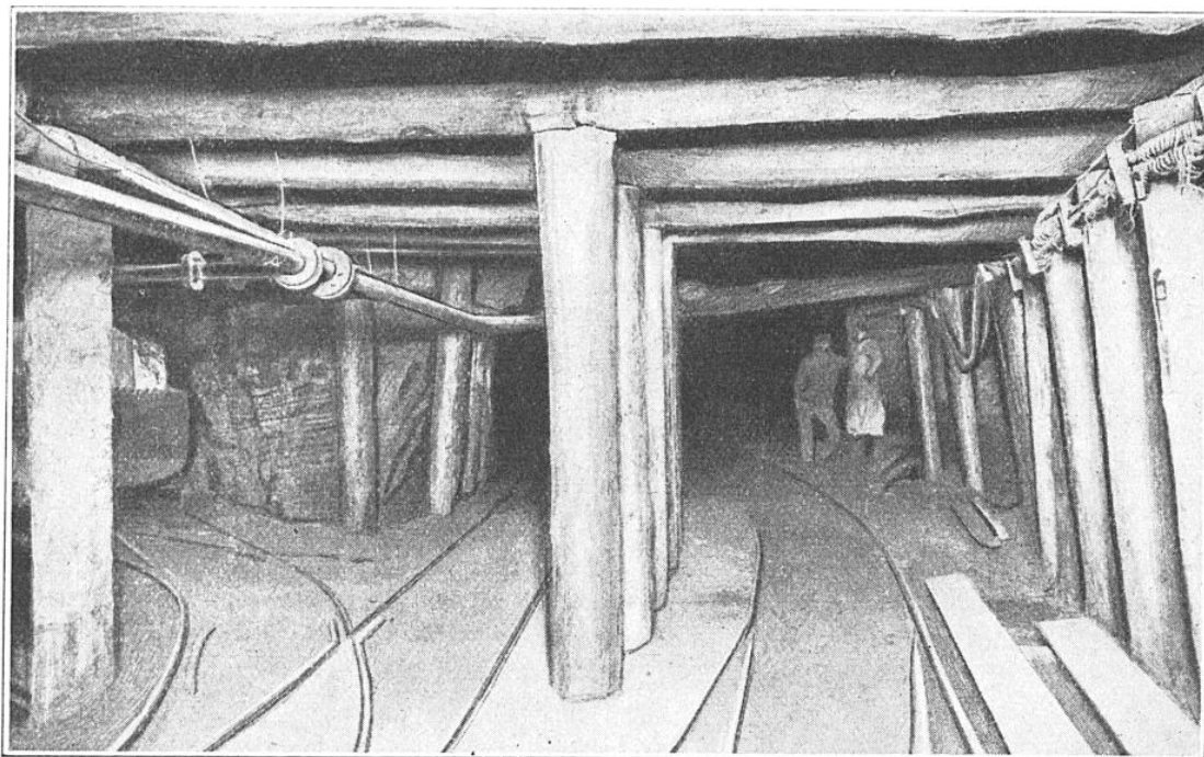
VUE D'UNE GALERIE PRINCIPALE D'EXPLOITATION DANS UNE MINE DE POTASSE
