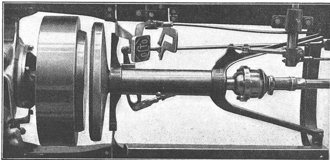
VUE EN PLAN DU CHANGEMENT DE VITESSE PAR SURFACES DE FRICTION
