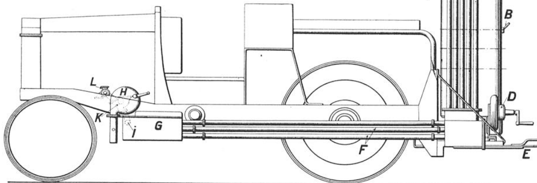
SCHÉMA DE MONTAGE DU GAZOGÈNE A BOIS SUR UN TRACTEUR AGRICOLE
