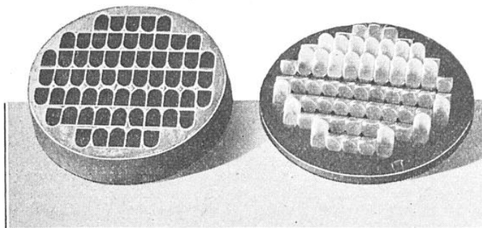
BLOCS DE PRISMES. PRÊTS POUR LE POLISSAGE
