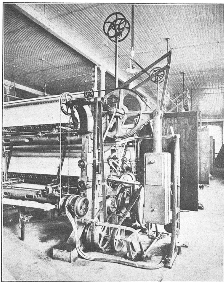
VUE PARTIELLE, FACE ARRIÈRE, DU MÉTIER PLAUEN
