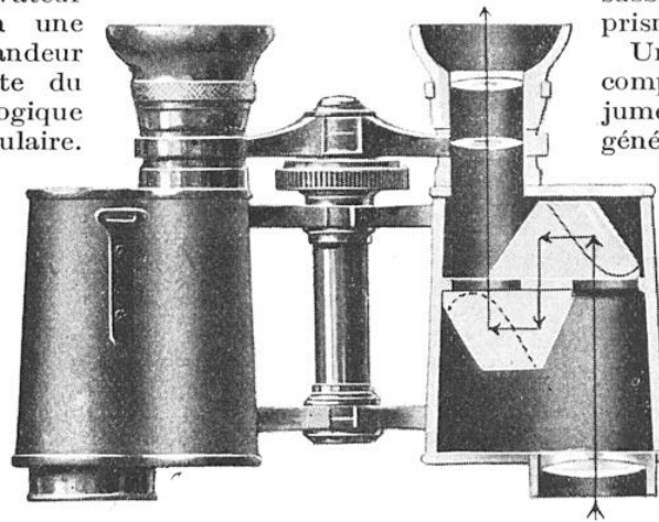
JUMELLE DEMI-COUPÉE MONTRANT LA MARCHÉ DES RAYONS LUMINEUX
