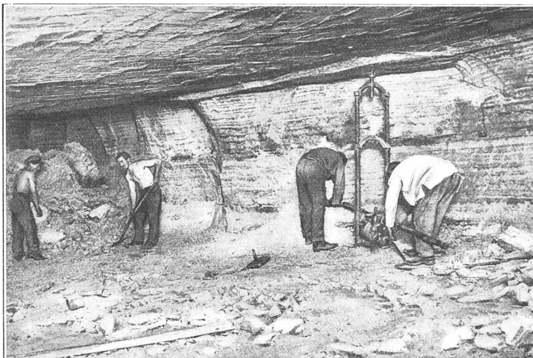
FORAGE D'UN TROU DE MINE A L'AIDE D'UNE PERFORATRICE A AIR COMPRIMÉ
