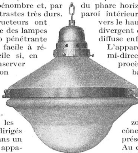
DIFFUSEUR POUR ÉCLAIRAGE DEMI-INDIRECT
