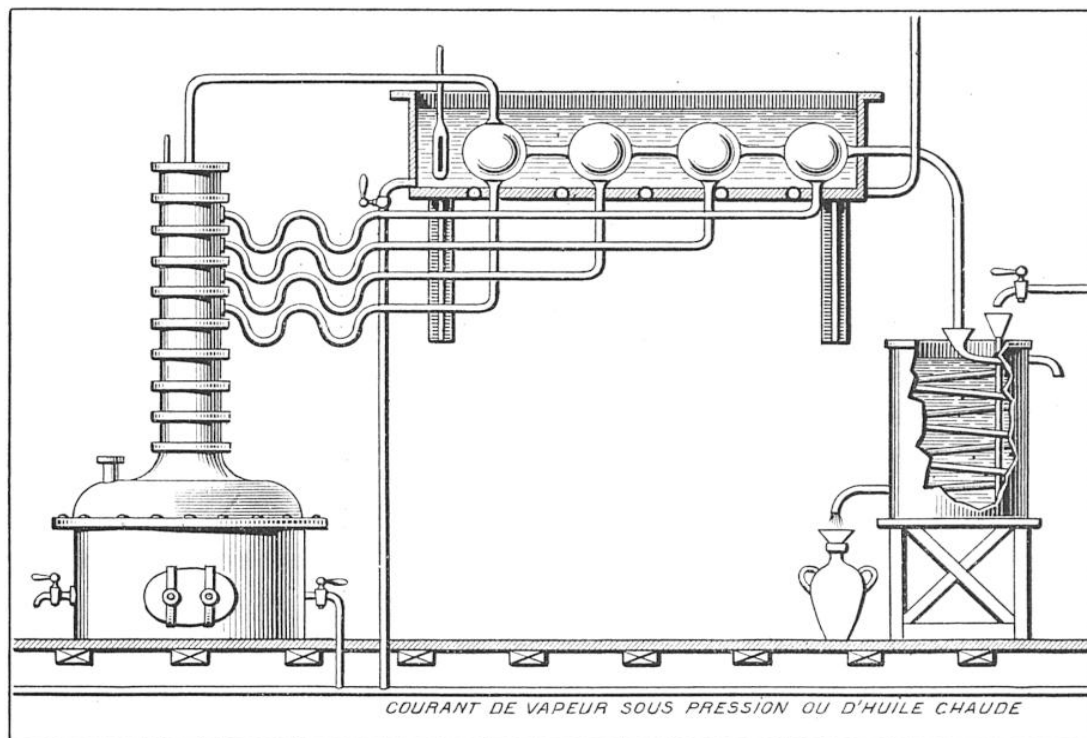
ALAMBIC CONSTRUIT POUR LE RAFFINAGE DU CAMPBRE, VU EN ÉLÉVATION
