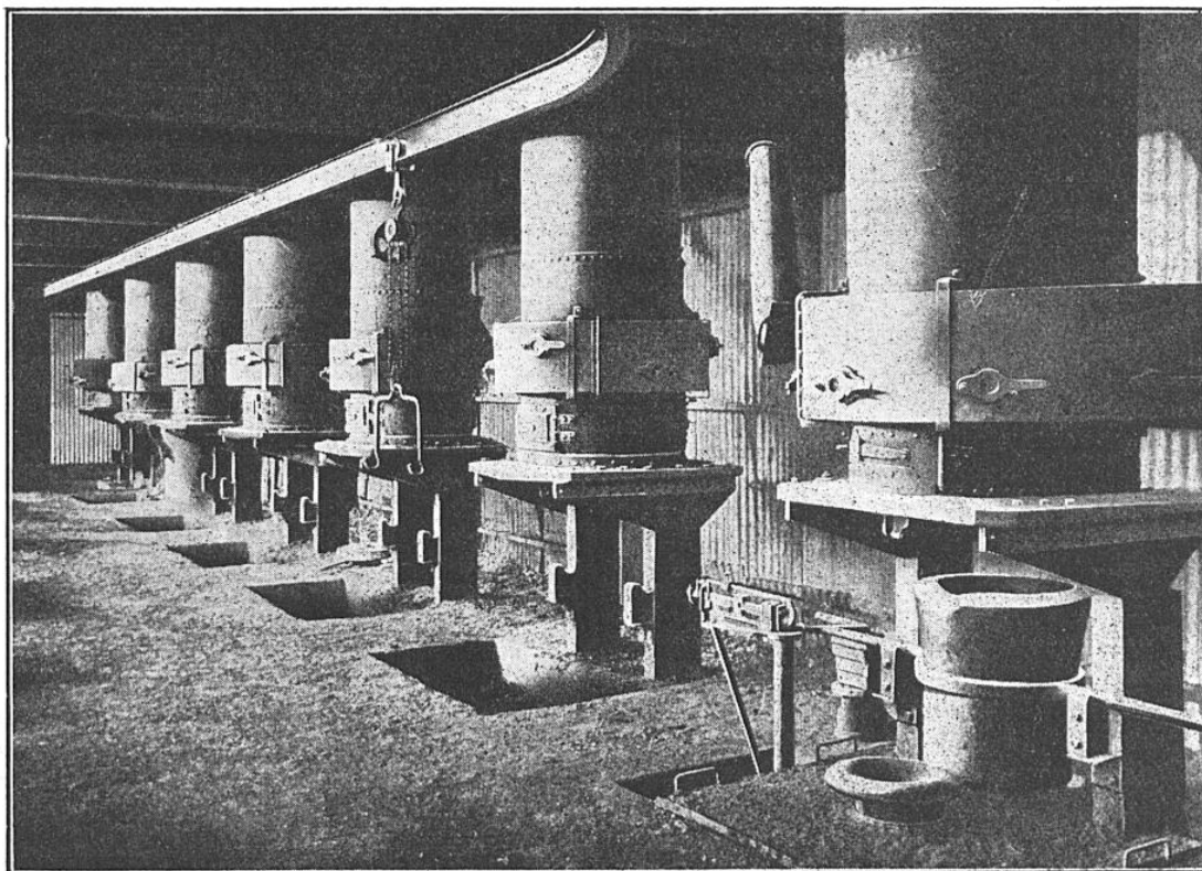
FIG. 4. — FOURS SERVANT A FONDRE LA FONTE POUR LA FABRICATION DES TUYAUX La fonte en fusion est recueillie dans des poches de coulée (dont une est visible au premier plan) et transportée ensuite dans les appareils d'alimentation des moules métalliques rotatifs.
