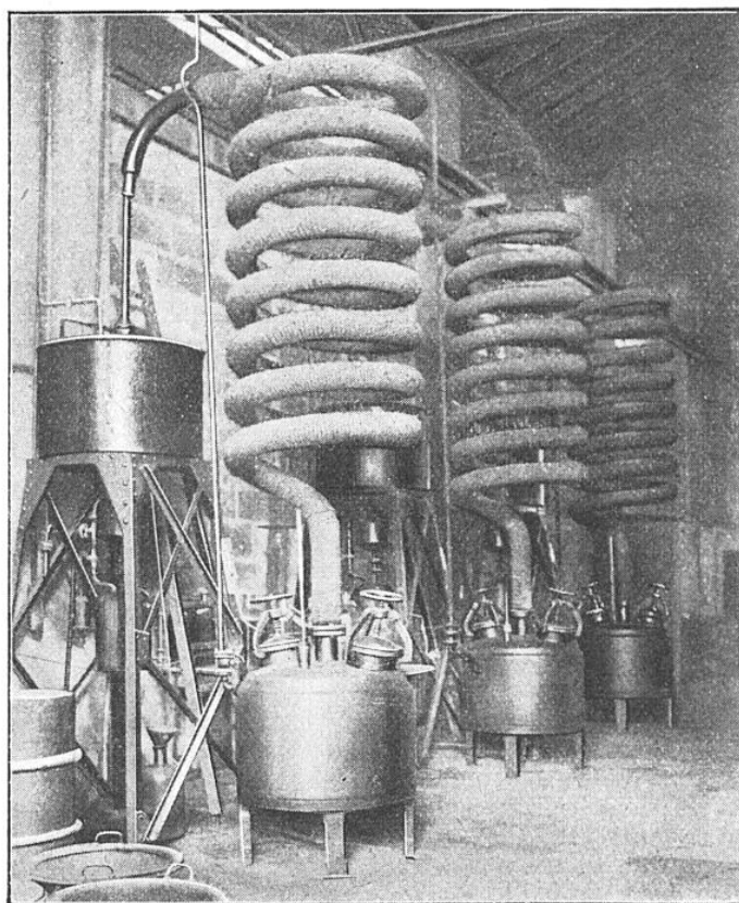
APPAREIL A DISTILLER DANS LE VIDE AVEC COLONNE-SERPENTIN CALORIFUGÉE
