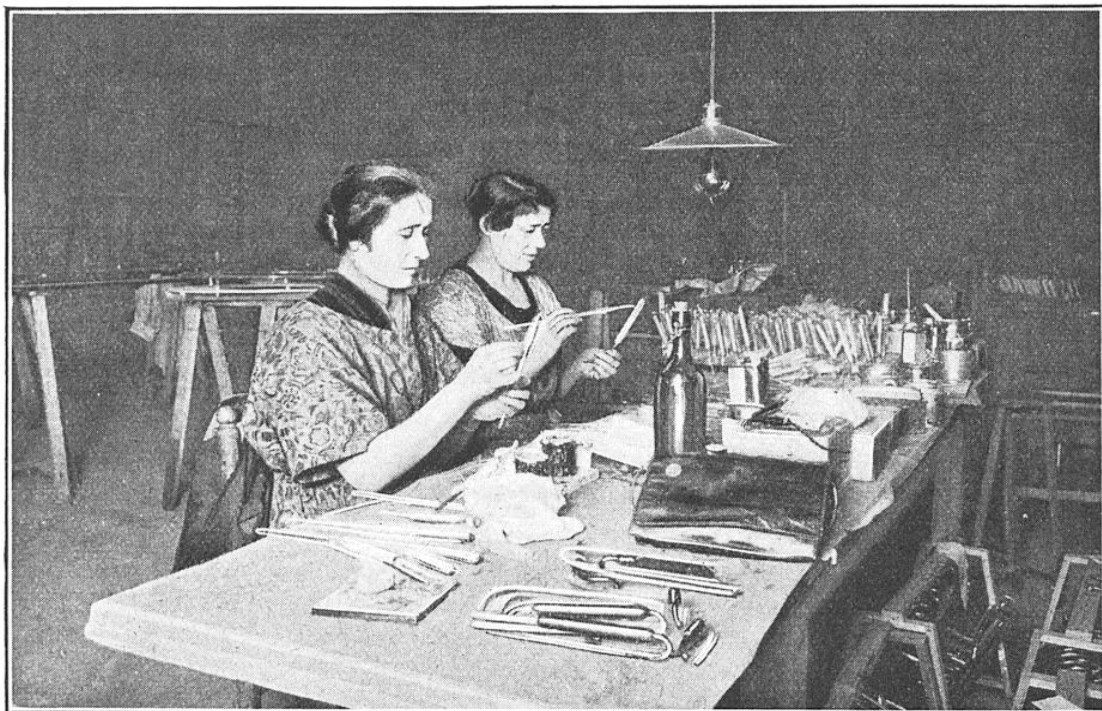
FIG. 2. — ATELIER DE PRÉPARATION DES PETITS TUBES LUMINESCENTS
