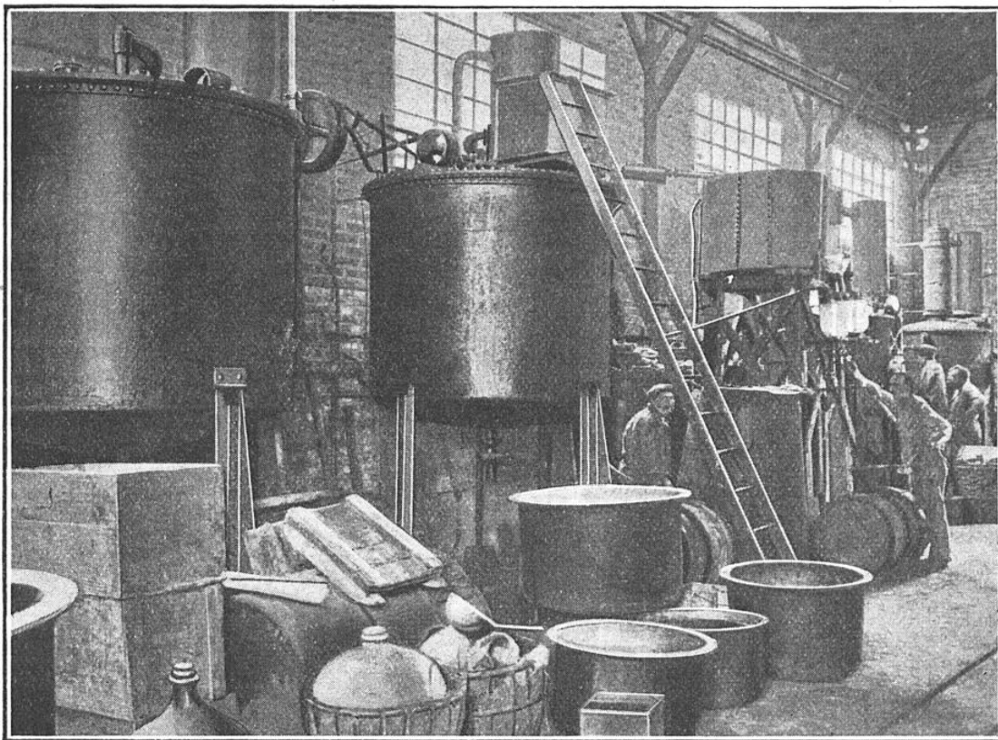
INSTALLATION POUR LA FABRICATION DU CYANURE DE BENZYLE
