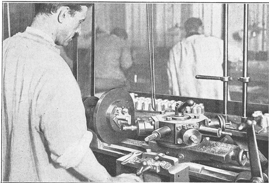
TOUR-REVOLVER MONTÉ POUR L'USINAGE DU CORPS DE JUMELLE
