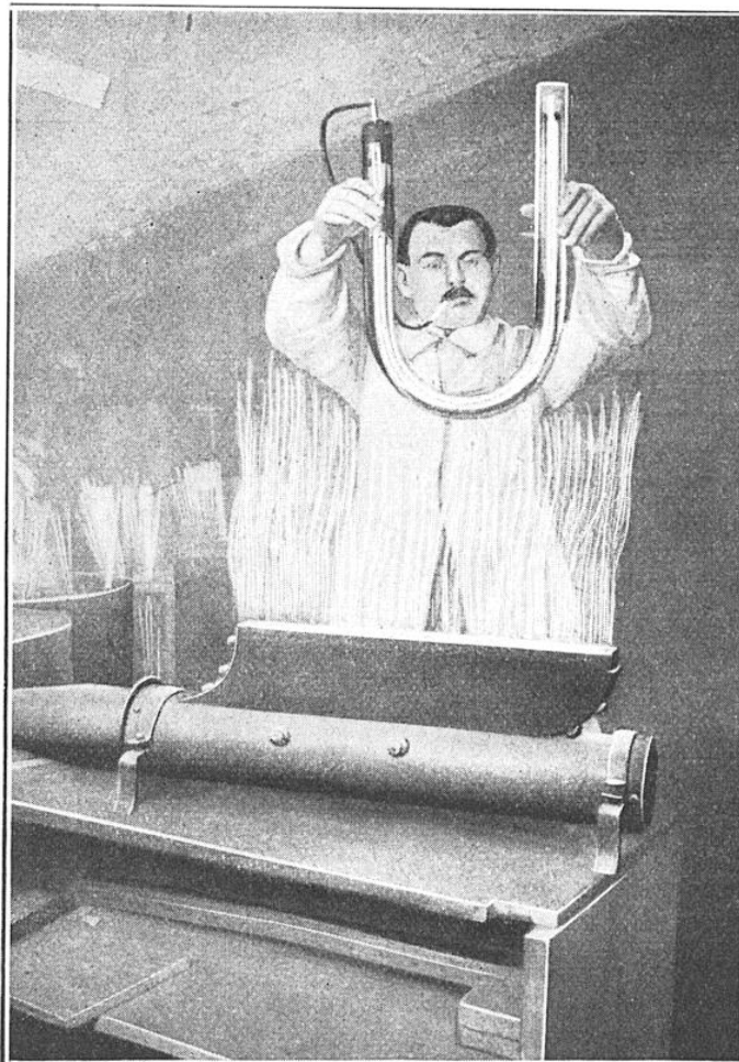
FIG. 3. — LES GROS TUBES SONT COURBÉS A LA MAIN DANS LA FLAMME D'UN ÉNORME « BUNSEN »
