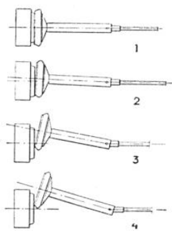
JEU DE LA COURONNE 1, prise directe ; 2, position intermédiaire ; 3, petite vitesse ; 4, marche arrière.
