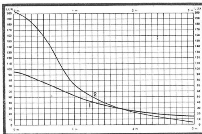
1 Lampe à incandescence sans appareil d'éclairage 2 Lampe avec appareil d'éclairage „URANUS“
