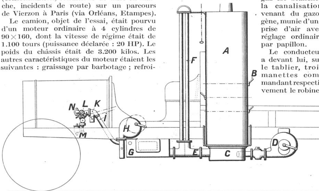
SCHEMA DE MONTAGE D'UN GAZOGENE A BOIS SUR UN CAMION
