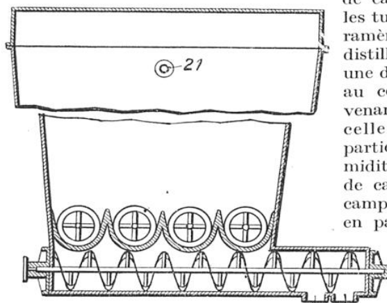
COUPE VERTICALE DU CONDENSEUR DE L'APPAREIL DU PONT DE NEMOURS
