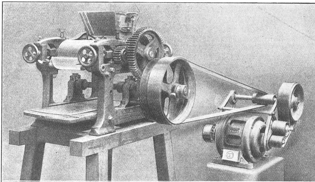
MOTEUR ÉLECTRIQUE ENTRAÎNANT UN BROYEUR AU MOYEN DU RÉDUCTEUR SOUPLE.
