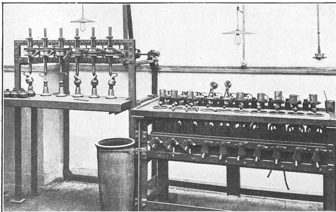
MACHINE A POLIR LES VERRES D'OCULAIRES ET DE PETITS OBJECTIFS
