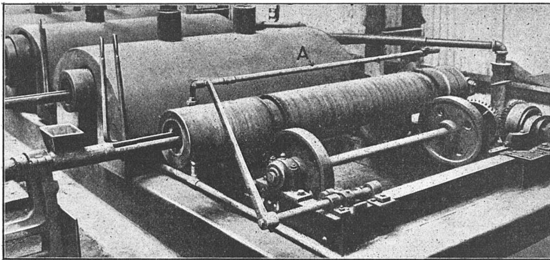
FIG. 3. — MACHINE BRÉSILIENNE PRIMITIVE POUR EXÉCUTER LA COULÉE ROTATIVE On remarque la rampe supérieure d'arrosage A destinée à remplir la chemise d'eau qui entoure le moule et à assurer le refroidissement du moule métallique. Dans la position de la photographie, le distributeur, constitué par une auge mobile et basculante, est à moitié engagé dans le moule.
