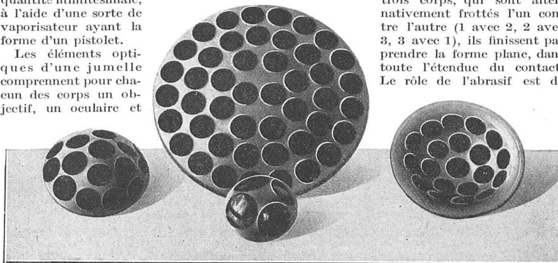
BLOCS DE LENTILLES POUR OBJECTIFS DISPOSÉES POUR LE POLISSAGE
