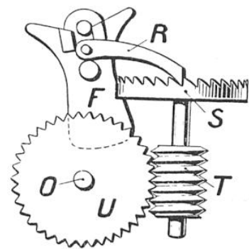
MÉCANISME D'ENTRAÎNEMENT DES AIGUILLES
