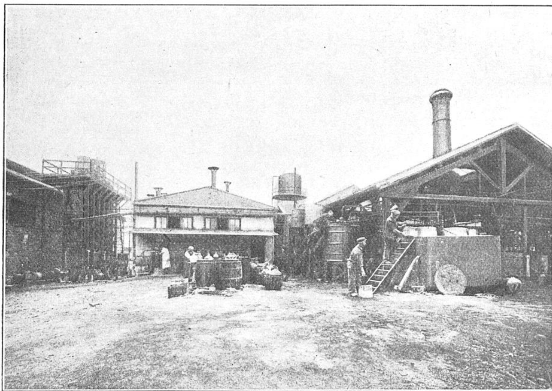
FABRICATION DU CHLORURE DE BENZYLE ET DE L'ALCOOL BENZYLIQUE DANS UNE IMPORTANTE USINE DES ENVIRONS DE PARIS
