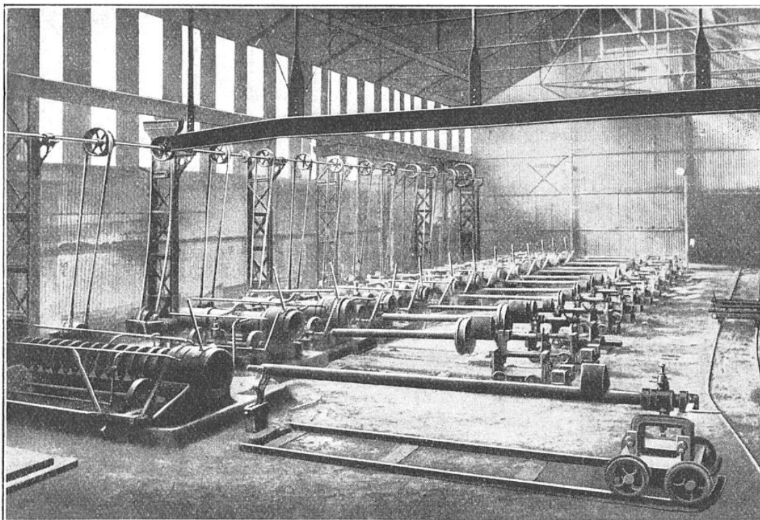
FIG. 2. — VUE, SOUS UN AUTRE ASPECT, DE LA BATTERIE DE MOULES MÉTALLIQUES REPRÉSENTÉE PAR LA FIGURE DE LA PAGE PRÉCÉDENTE
