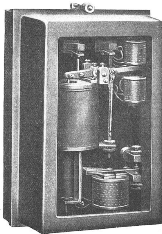
FIG. 14. — VOLTMÈTRE A CONTACTS PROVOQUANT AUTOMATIQUEMENT LA MISE EN MARCHÉ OU L'ARRÊT D'UNE CENTRALE AUTOMATIQUE
