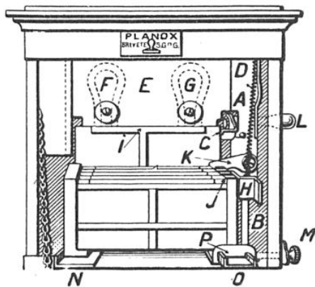
COUPE DU STÉRÉOSCOPE « PLANOX »
