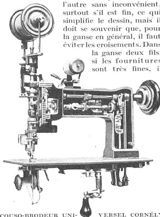
COUSO-BRODEUR UNI-VERSEL CORNÉLY
