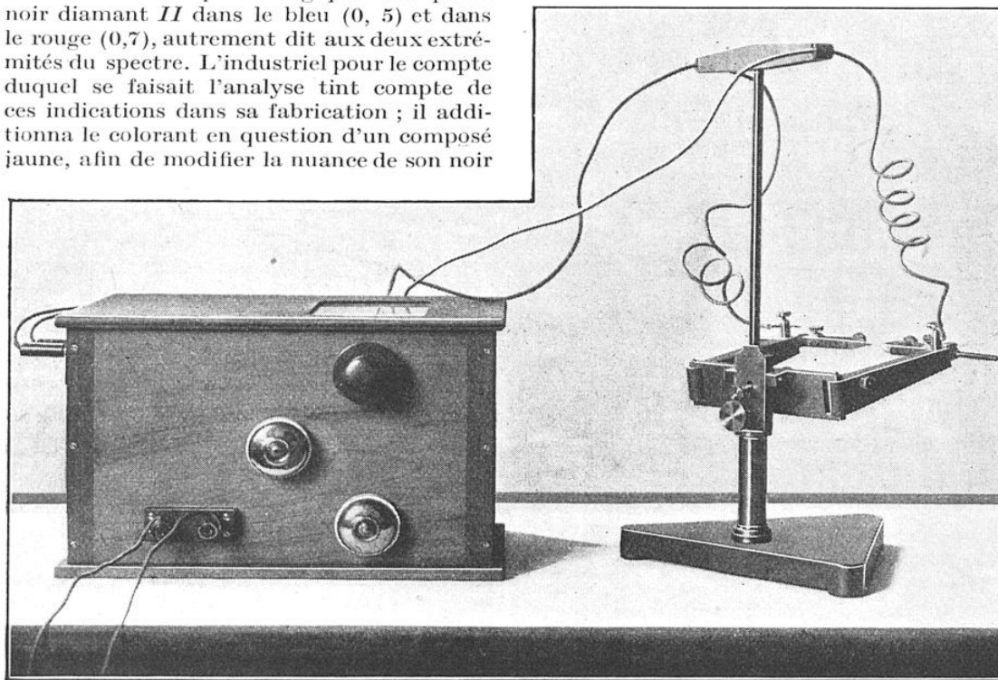
FIG. 9. — DISPOSITIF DE HAUTE FRÉQUENCE CAPABLE DE FOURNIR UNE ÉTINCELLE NOURRIE ET CHAUDE POUR L'EXAMEN SPECTROPHOTOMÉTRIQUE DES HUILES ESSENTIELLES
