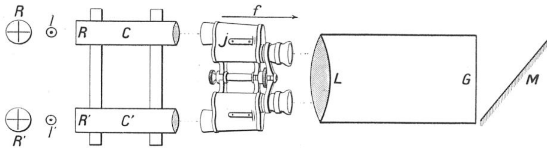
RÉGLAGE DU PARALLÉLISME DES AXES DES DEUX CORPS DE LA JUMELLE
