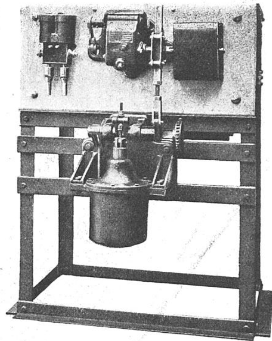
FIG. 5. — UN AUTRE INTERRUPTEUR COMMANDÉ À DISTANCE
