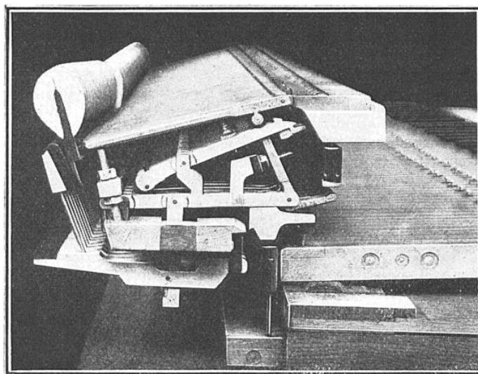
VUE DE COTÉ, A GRANDE ÉCHELLE, D'UNE AUTRE PARTIE DE LA MÉCANIQUE SPÉCIALE ÉTUDIÉE PAR LA MAISON PLEYEL POUR LA RÉALISATION DU DOUBLE CLAVIER HANS
