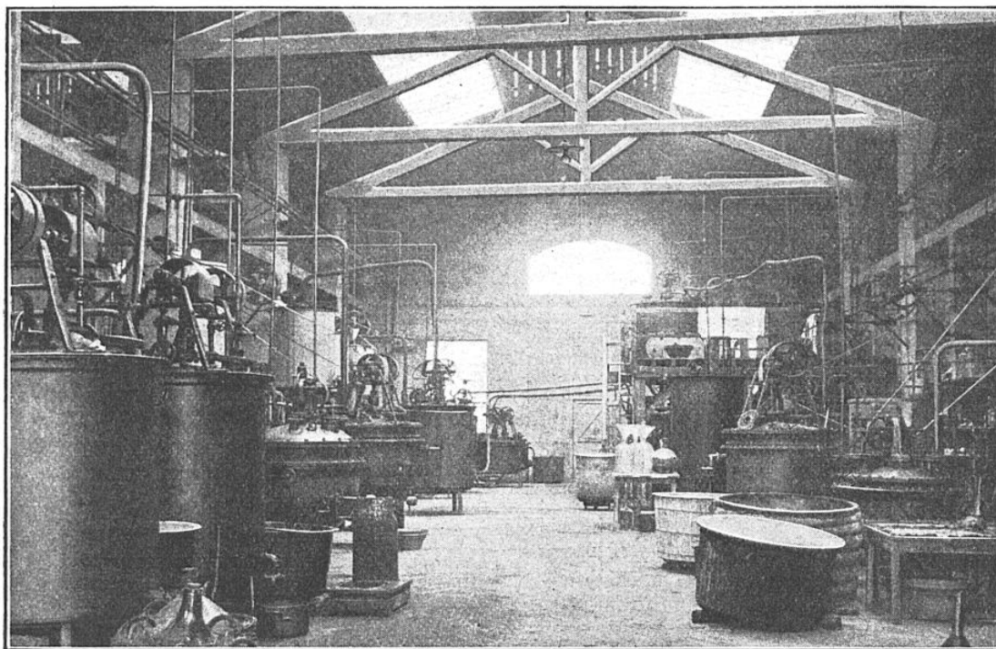
APPAREILS A RÉACTION AVEC RÉFRIGÉRANT DESCENDANT POUR LA FABRICATION D'ALCOOL PHÉNYLÉTHYLIQUE, DE TERPINÉOL ET DE DIVERS ÉTHERS
