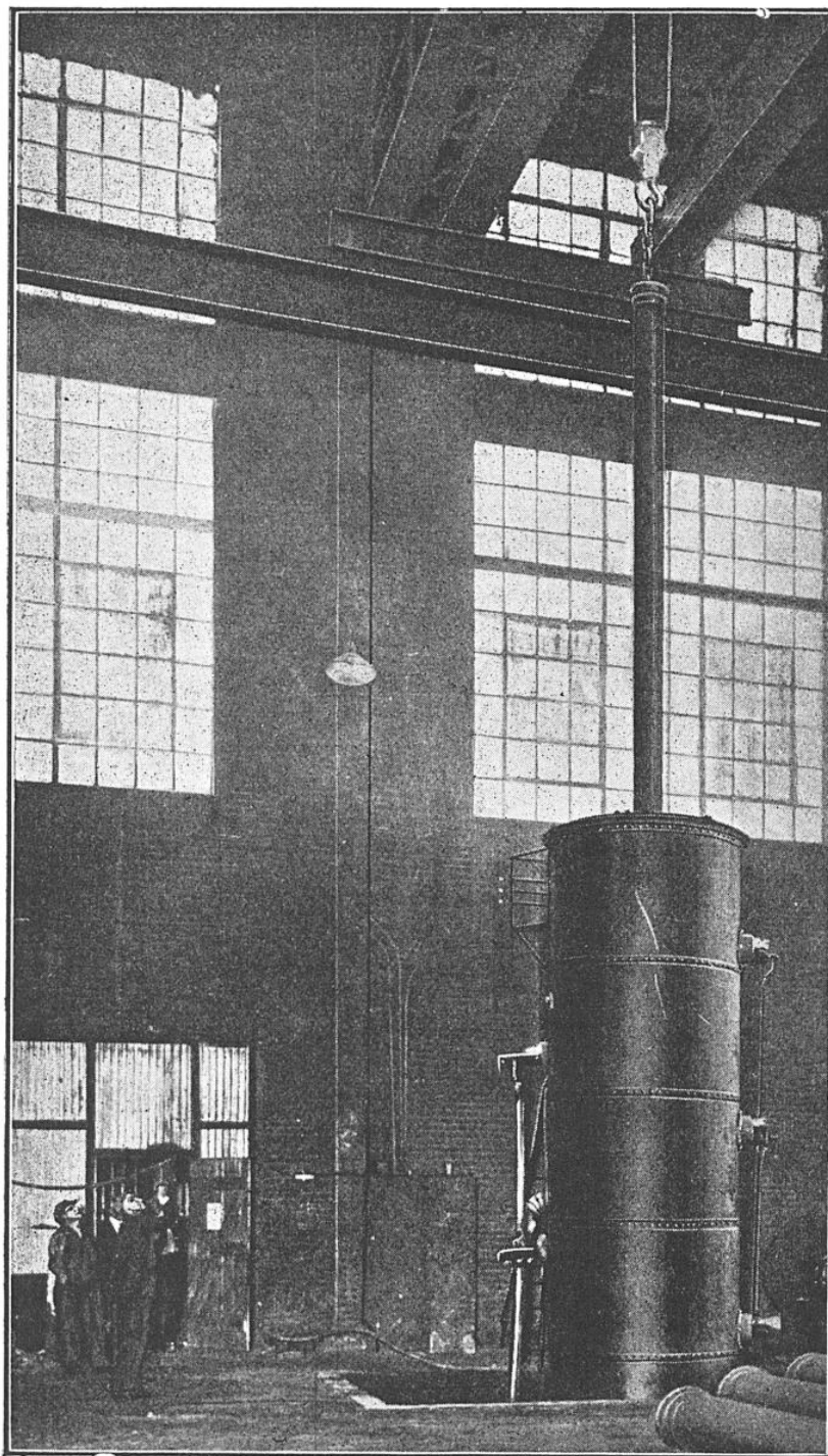
FIG. 16. — RÉCHAUFFAGE D'UN TUYAU IMMÉDIATEMENT APRÈS SA SORTIE DU MOULE ROTATIF
