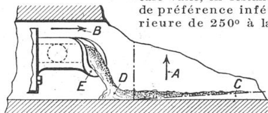
FIG. 14. — FORMATION D'UN TUYAU PAR LE PROCÉDÉ DE LA COULÉE ROTATIVE
