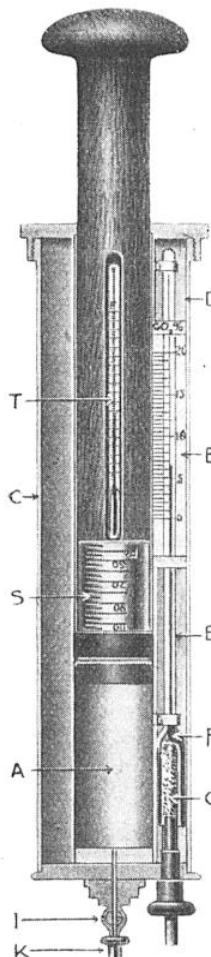
VUE EN COUPE DU THERMOSCOPE
