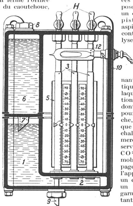
VUE EN COUPE DU MANOMÈTRE « SAFA »
