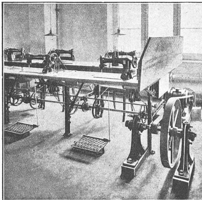
BANC DE COUSO-BRODEURS ACTIONNÉS PAR UN MOTEUR ÉLECTRIQUE SYSTÈME OERLIKON
