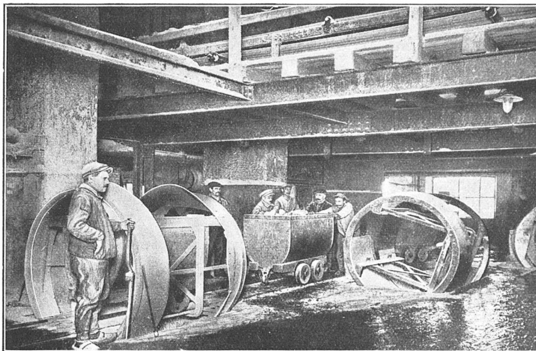
CULBUTEURS SERVANT A BASCULER LES WAGONNETS SORTANT D'UN PUIT CHARGÉS DE MINÉRAI POTASSIQUE, DANS UNE MINE D'ALSACE
