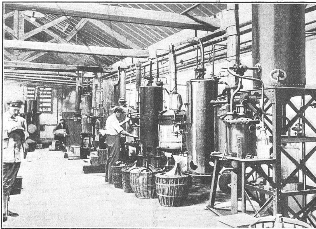
APPAREILS A RECTIFIER DANS LE VIDE POUR LA FABRICATION DU PARFUM DE VIOLETTE ARTIFICIEL PAR LES PROCÉDÉS CHIMIQUES
