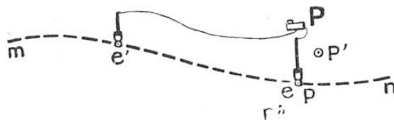
FIG. 5. — DISPOSITIF THÉORIQUE POUR LA RECHERCHE DES COURBES ÉQUIPOTENTIELLES. L'électrode e' étant placée sur la courbe m n , l'aiguille du potentiomètre se déplacera à droite si l'on touche, avec l'électrode e , des points p' situés d'un certain côté de m n , à gauche, pour un contact en p'' et restera immobile en p sur la courbe.
