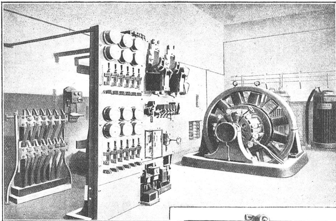
FIG. 13. — USINE ÉLECTRIQUE FONCTIONNANT AUTOMATIQUEMENT
