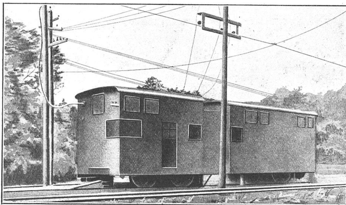
FIG. 3. — N'AYANT AUCUN PERSONNEL, CETTE SOUS-STATION AUTOMATIQUE ROULANTE PEUT ÊTRE PLACÉE EN UN ENDROIT QUELCONQUE, MÊME ÉLOIGNÉ DE TOUT CENTRE HABITÉ
