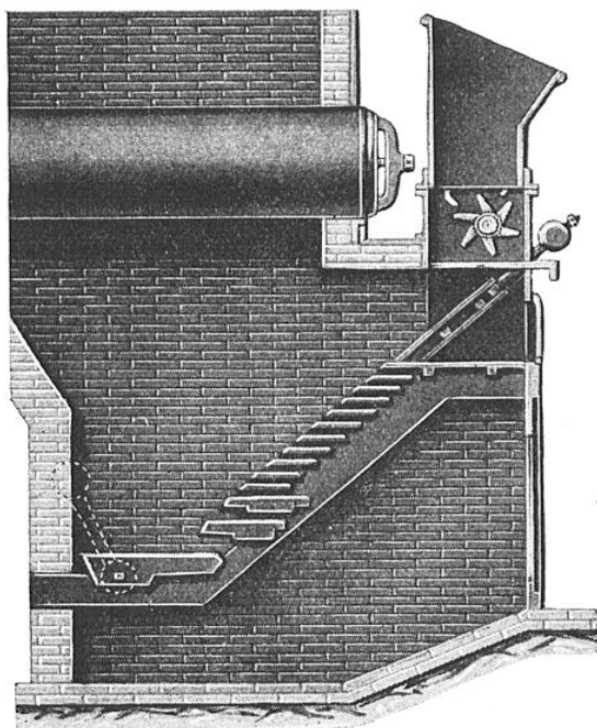
FOYER MARGO POURVU D'UNE INSTALLATION D'ALIMENTATION AUTOMATIQUE
