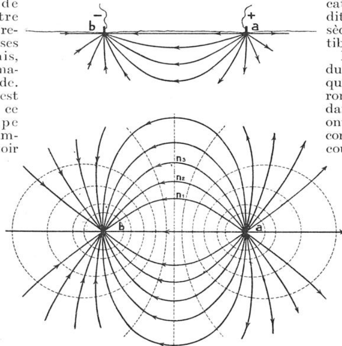
FIG. 2.— PERTURBATIONS ÉLECTRIQUES AUTOUR DE DEUX PRISES DE TERRE a ET b EN TERRAIN HOMOGÈNE
