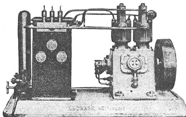
Compresseur à haute pression, 150 kgs par \text{cm}^2 .
