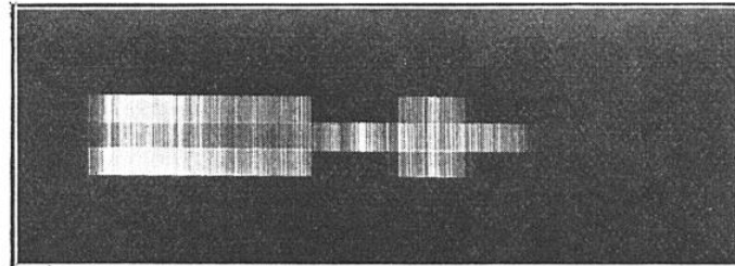
FIG. 11. — SPECTROPHOTOGRAMMES RELATIFS A DEUX SOLUTIONS TRÈS DILUÉES D'ESSENCE D'ANIS
