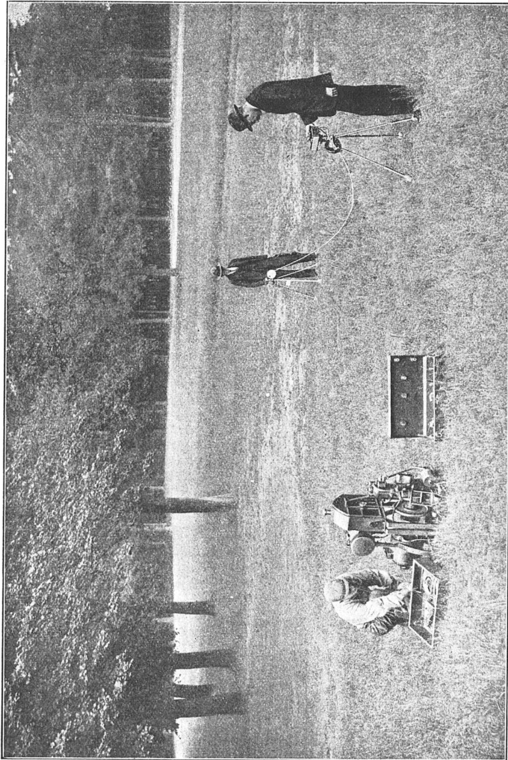
VUE PRISE SUR LES MORTS-TERRAINS RECOUVRANT UN GISEMENT MÉTALLIFÈRE DONT ON CHERCHE À PRÉCISER L'EMPLACEMENT
