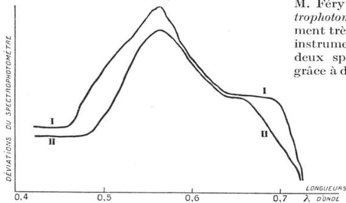
FIG. 5. — DIFFÉRENCIATION PAR LA MÉTHODE SPECTROPHOTOMÉTRIQUE DE DEUX PRODUITS TINCTORIAUX CONNUS SOUS LE NOM DE « NOIRS DIAMANTS »
