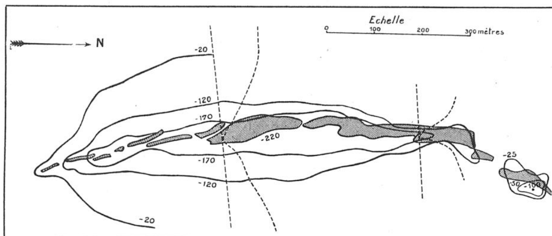
FIG. 9. — CARTE DE POLARISATION SPONTANÉE DES CÉLÈBRES AMAS DE PYRITE DE « SAIN-BEL », SITUÉS DANS LE DÉPARTEMENT DU RHONE
