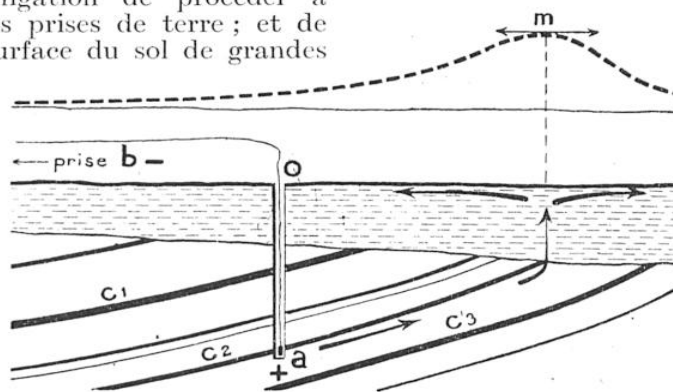
FIG. 14. — ÉTUDE DU PENDAGE OU INCLINAISON. D'UNE FORMATION HOUILLÈRE A L'AIDE D'UN SONDAGE C 1 C 2 C 3 , couches de houille. Le courant, canalisé entre ces couches, remonte à la surface à l'aplomb du point où la couche C 2 vient finir sous les morts-terrains. Il en résulte, en ce point, une bosse m caractéristique du profil des potentiels.
