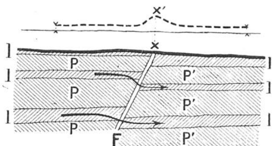
FIG. 12. — PASSAGE D'UNE FAILLE
