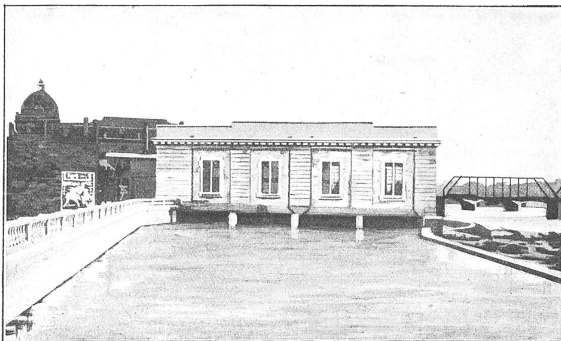
FIG. 16. — VUE DE LA SOUS-STATION ÉLECTRIQUE DE CEDAR-RAPIDS (ÉTATS-UNIS) Cette station a été installée au mois de décembre 1914 ; elle fonctionne absolument sans personnel. La commande automatique des machines est réalisée par le niveau de la rivière elle-même.
