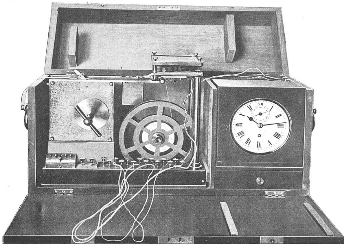
L'ÉLECTROCHRONOGRAPHIE DANS LA CAISSE QUI LE RENFERME
