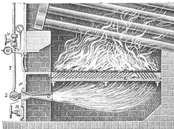
VUE EN COUPE D'UN FOYER MUNI D'UNE GRILLE POILLON AVEC SOUFFLERIE A VAPEUR P, plaque de fermeture du cendrier; R, porte pour enlever les cendres et mâchefers; S, bec d'arrivée de vapeur dans chaque tuyère; C, tuyère dont le nombre varie avec la surface de la grille et la quantité de charbon à brûler; T, tuyau d'arrivée de vapeur; V, valve de réglage de la vapeur de la soufflerie; E, traverses de support des barreaux.
