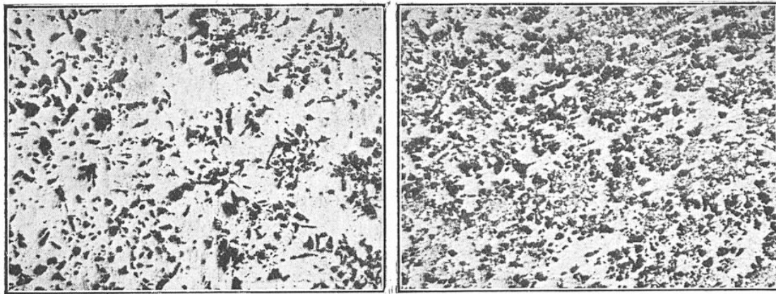
FIG. 15. — MICROPHOTOGRAPHIES MONTRANT LA DIFFÉRENCE EXISTANT ENTRE LES MÉTAUX OBTENUS, SUIVANT LA MÉTHODE DE COULAGE EMPLOYÉE
