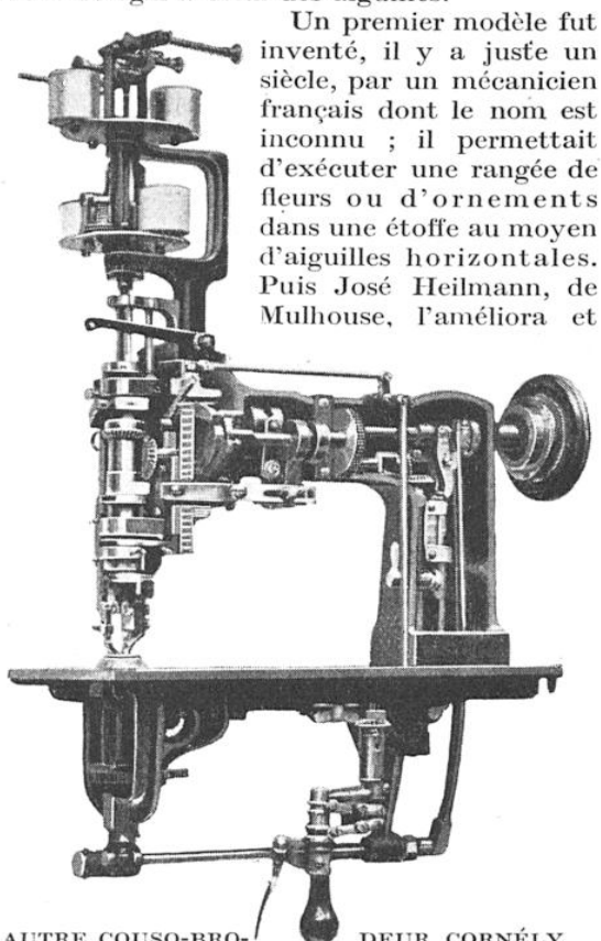
AUTRE COUSO-BRO- DEUR CORNÉLY Cette machine produit tous les effets à jour (point clair) en ligne droite, aussi bien que dans toutes les directions de la broderie.
