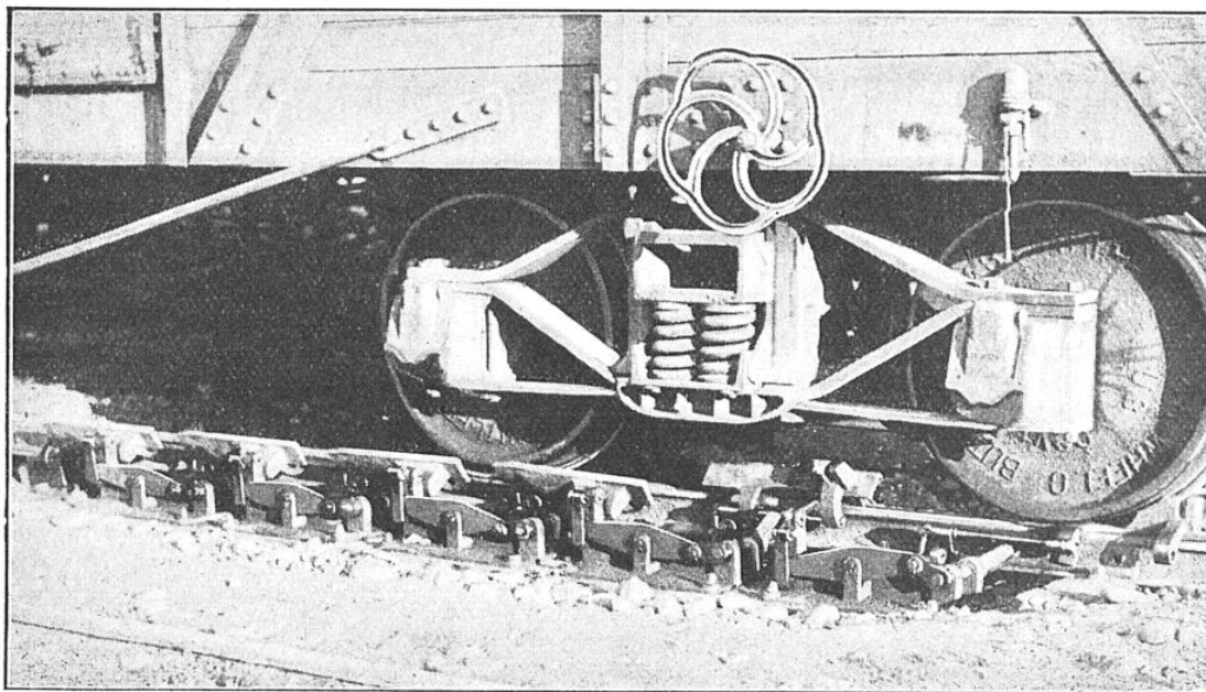
GROUPE DE SIX SABOTS-FREINS ARRÊTANT UN WAGON A BOGIE
