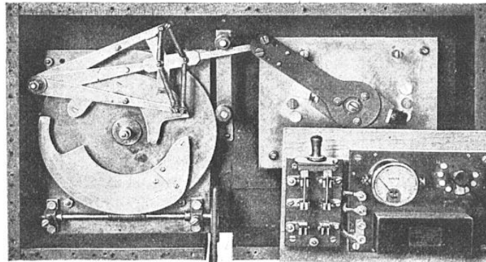
FIG. 15. — INVERSEUR AUTOMATIQUE DE COURANT
