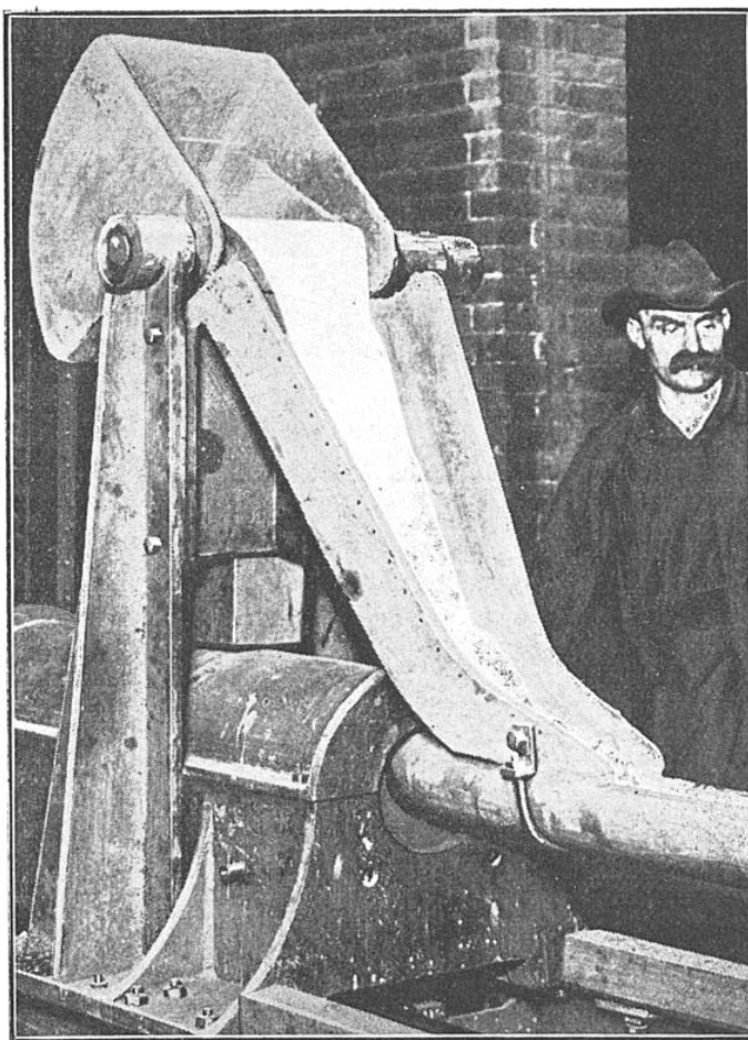
FIG. 11. - DISPOSITIF D'ALIMENTATION D'UN DISTRIBUTEUR La fonte en fusion est versée dans le réservoir supérieur. Au fur et à mesure que le moule s'éloigne, un piston hydraulique soulève ce réservoir qui déverse son contenu dans le distributeur.
