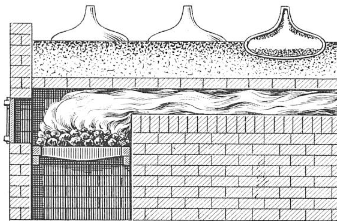
COUPE D'UN FOUR DE CHAUFFAGE A SABLE POUR LA SUBLIMATION DU CAMPHRE
