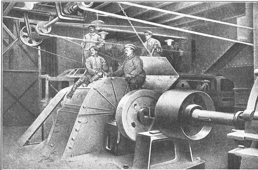
MOULIN MÉCANIQUE SERVANT À BROYER LA SYLVINITE (CHLORURE NATUREL DE POTASSIUM) PROVENANT D'UNE MINE DE POTASSE
