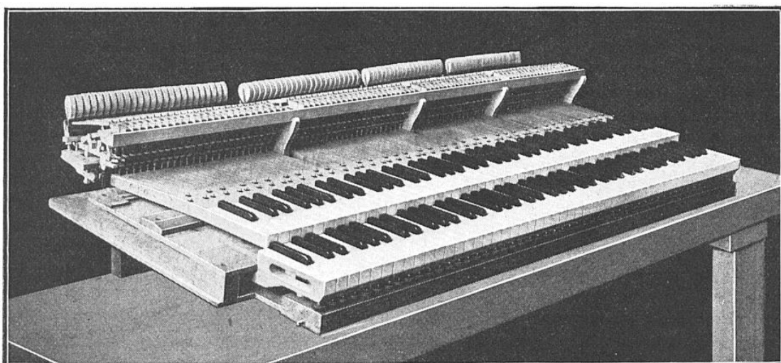
PHOTOGRAPHIE MONTRANT LA RÉALISATION DU DOUBLE CLAVIER HANS
