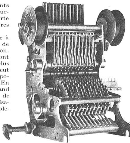
DÉTAIL DU MÉCANISME IMPRIMANT DE LA MACHINE À CALCULER
