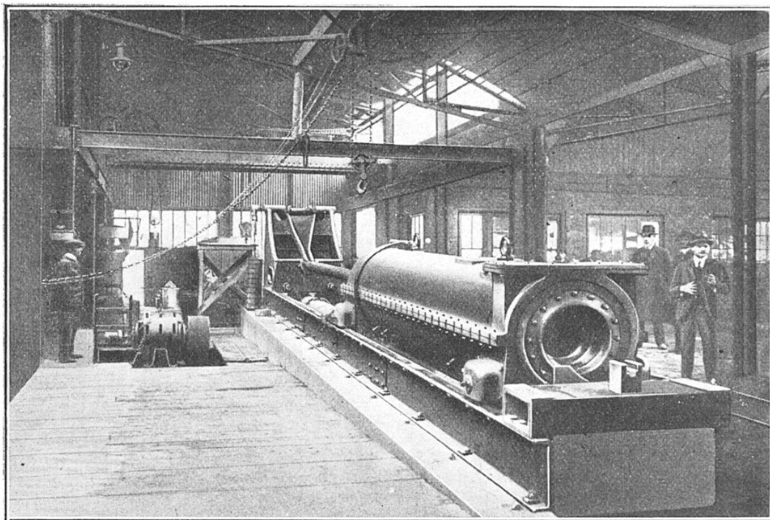
FIG. 7. — VUE DE LA MACHINE PERFECTIONNÉE DE M. D. S. DE LAVAUD POUR L'OBTENTION DES TUYAUX DE FONTE PAR COULÉE ROTATIVE
