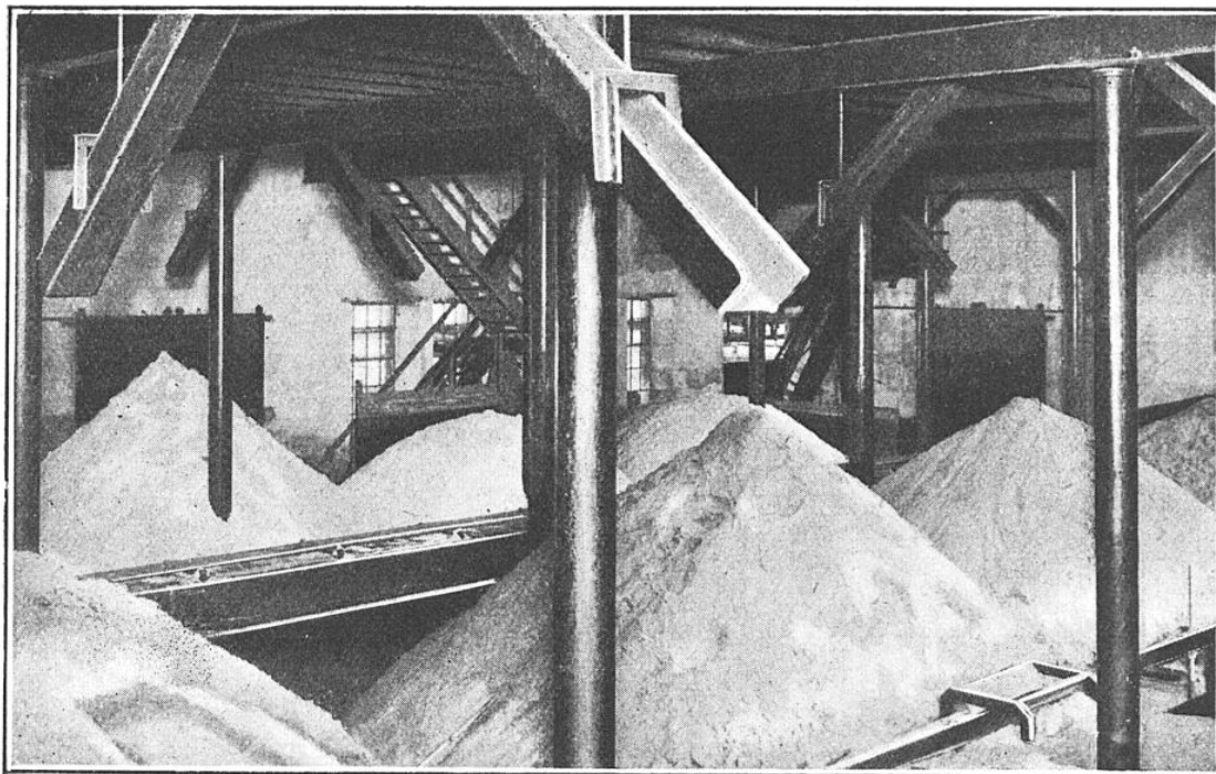
MISE EN TAS DU CHLORURE DE POTASSIUM AU MOYEN DE GOULOTTES
