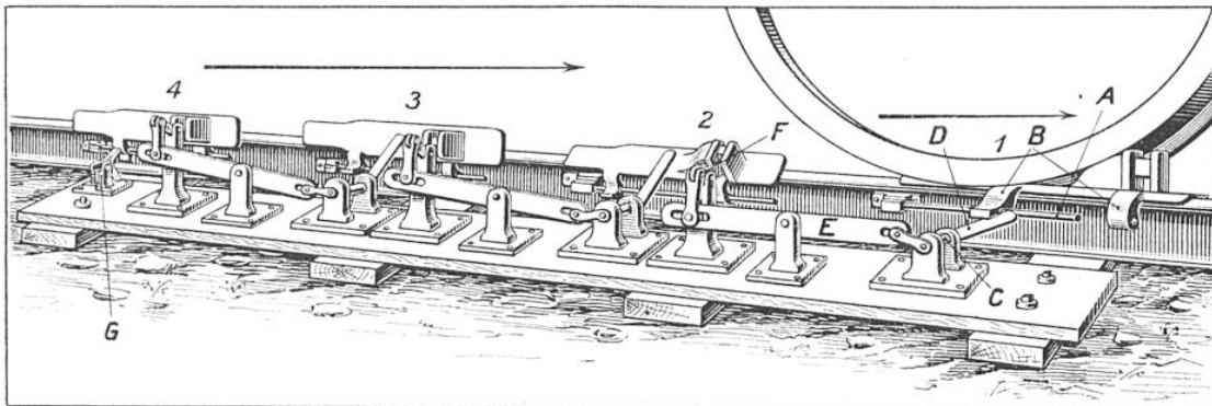
MÉCANISME DU SYSTÈME DE SABOTS-FREINS IMAGINÉ PAR M. CHASSY
