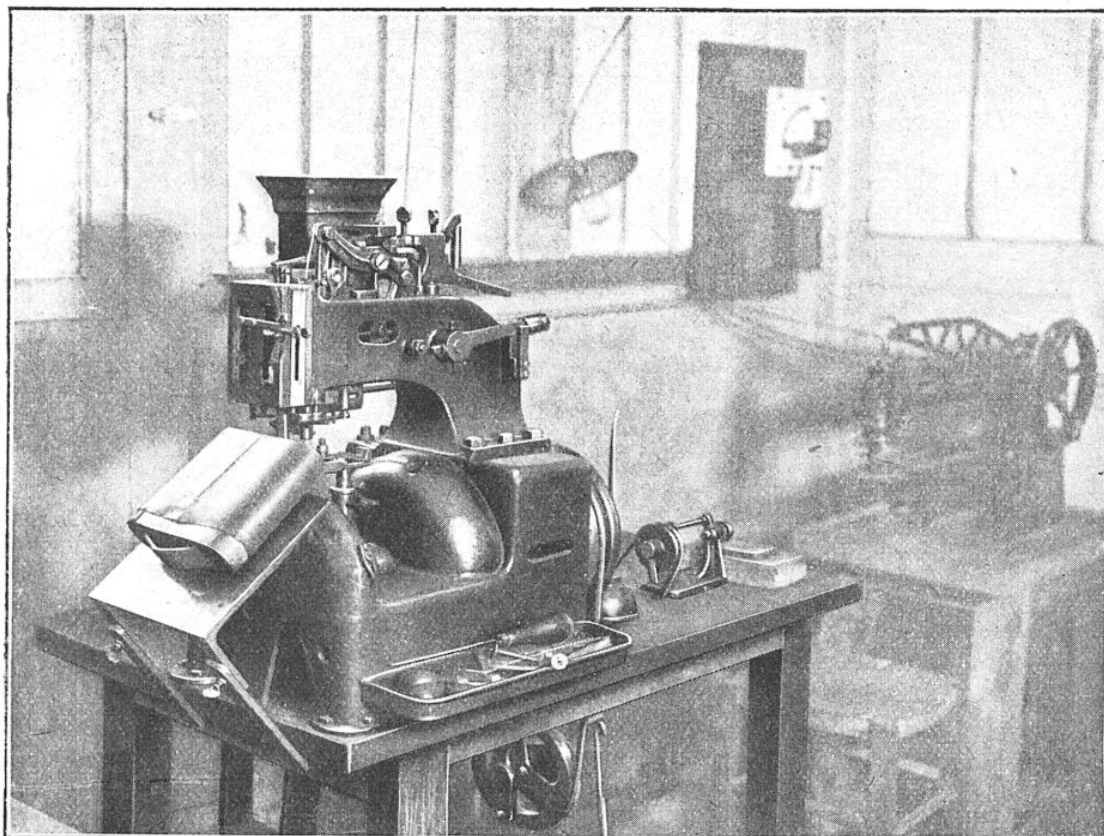
MACHINE SPÉCIALE COUSANT LES ÉTUIS A JUMELLES EN CUIR
