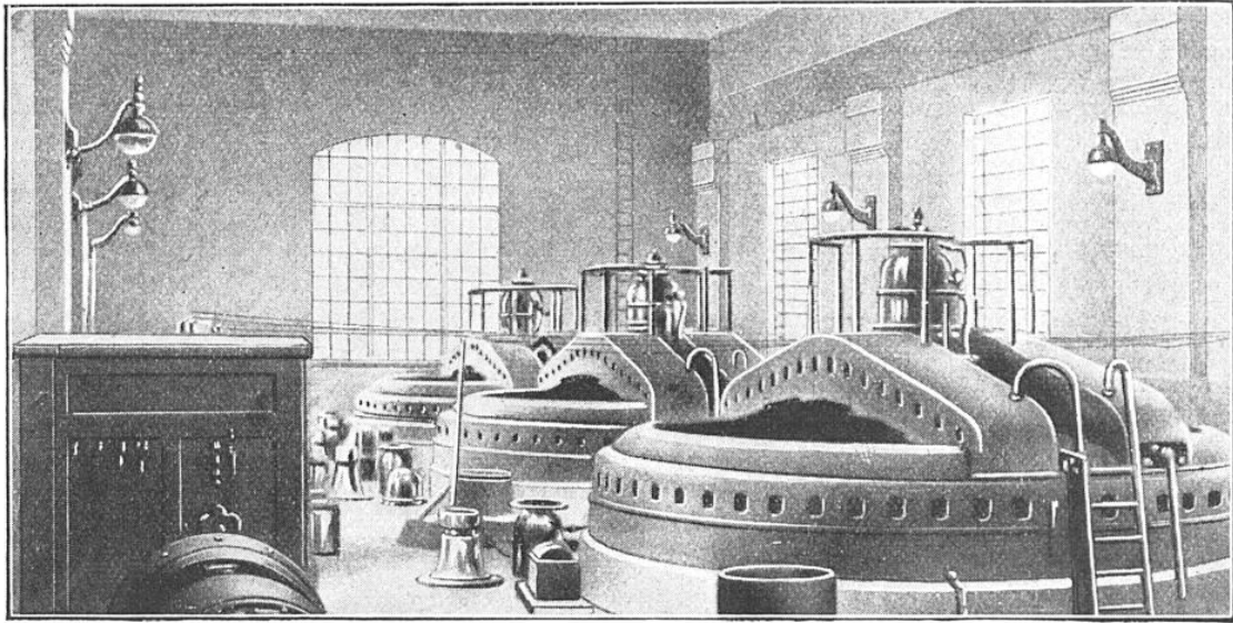
FIG. 17. — VUE INTÉRIEURE DE L'USINE AUTOMATIQUE DE CEDAR-RAPIDS
