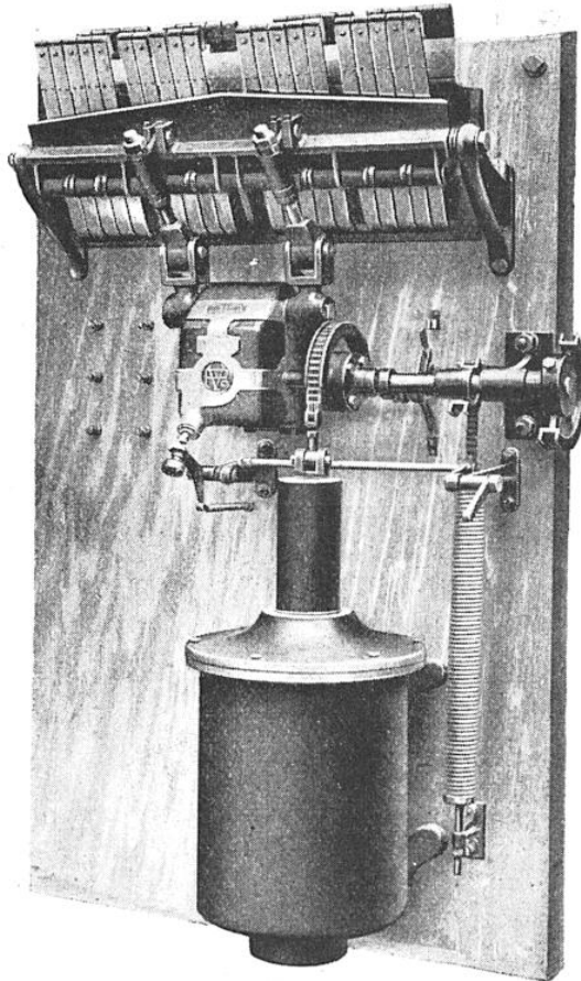
FIG. 4. — UN ÉLECTRO-AIMANT, ACTIONNÉ PAR UN COURANT LANCÉ D'UN POINT TRÈS ÉLOIGNÉ, OUVRE OU FÈRME À VOLONTÉ LE CIRCUIT DU GROS INTERRUPTEUR PLACÉ EN HAUT
