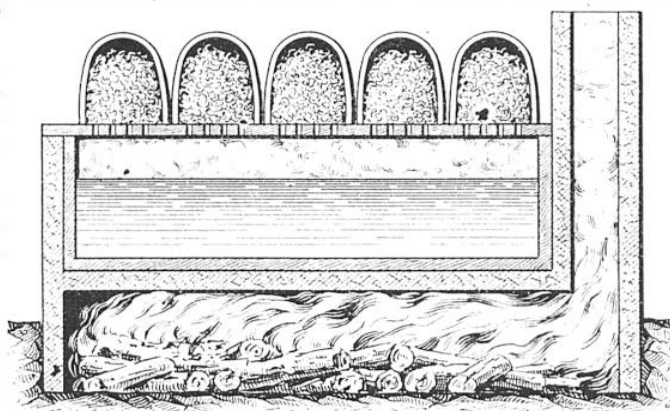
COUPE DU FOURNEAU EMPLOYÉ DANS LES FORÊTS DE L'ÎLE DE FORMOSE POUR LA SUBLIMATION DU CAMPBRE
