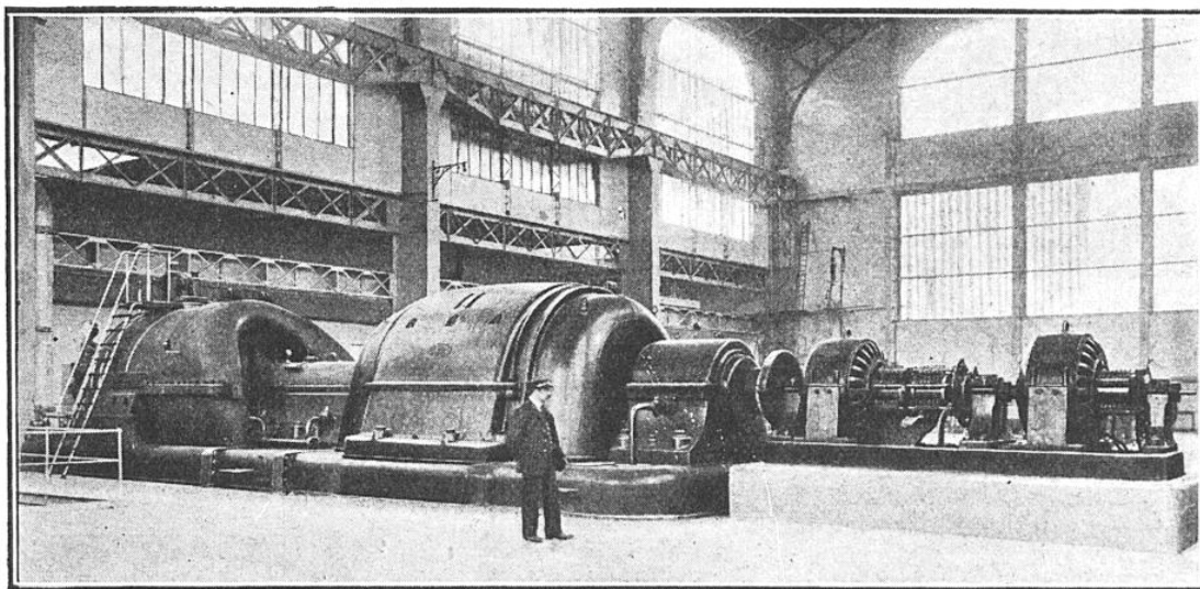
FIG. 1. — PAR SUITE DE L'APPLICATION DES DISPOSITIFS AUTOMATIQUES DE RÉGLAGE, LES USINES MODERNES FONCTIONNENT AVEC UN PERSONNEL TRÈS RESTREINT
