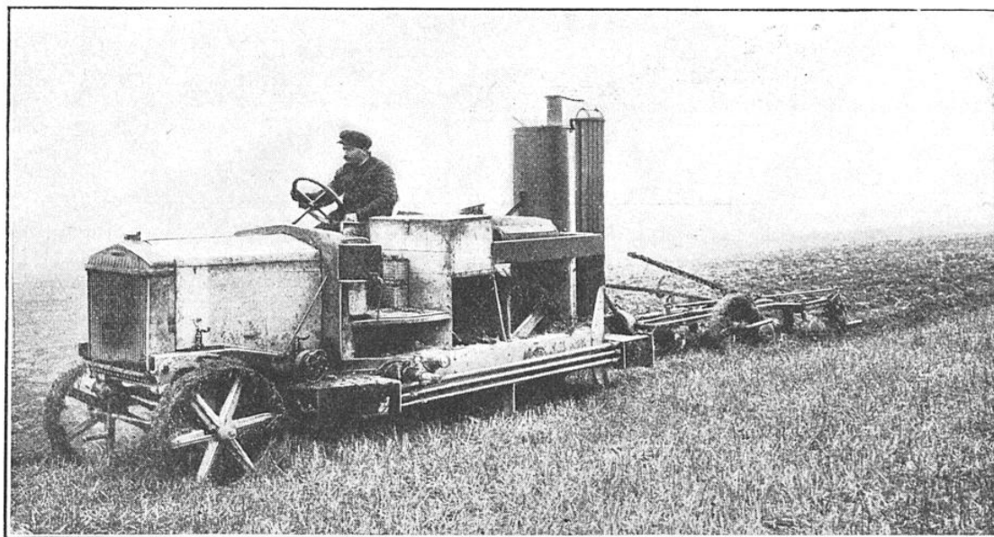
TRACTEUR AGRICOLE MARCHANT AU GAZ PAUVRE, AVEC GAZOGÈNE A BOIS
