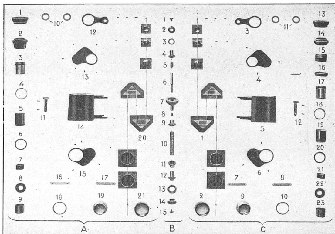
LES PRINCIPALES PIÈCES MÉTALLIQUES ET D'OPTIQUE NÉCESSAIRES AU MONTAGE D'UNE JUMELLE A PRISMES A MISE AU POINT SIMULTANÉE
