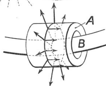
CHAMP MAGNÉTIQUE DE L'AIMANT SPÉCIAL
