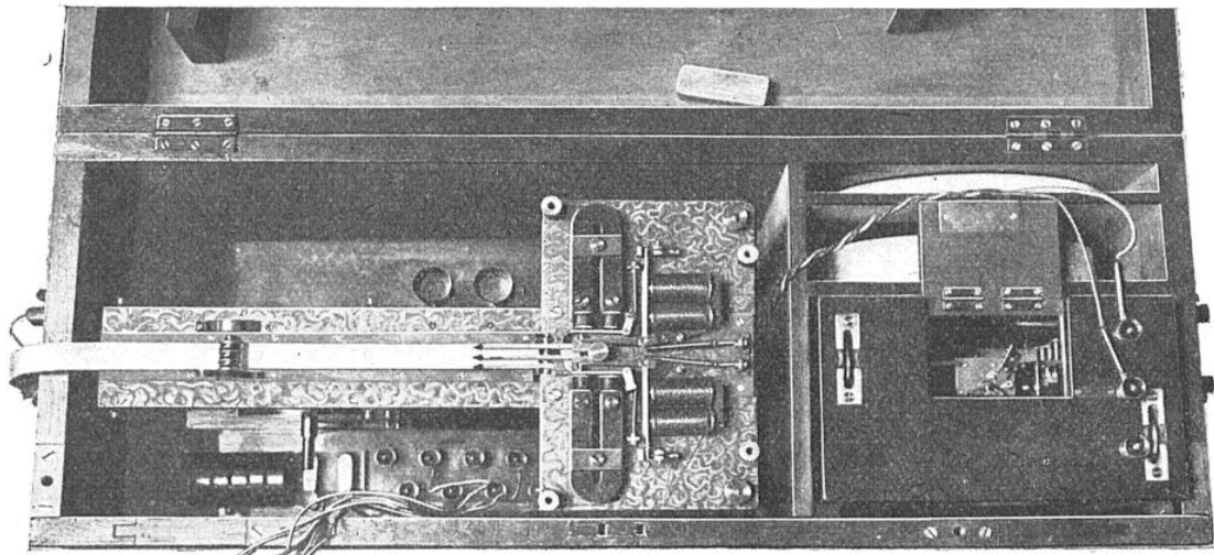
VUE PAR DES- SOUS DE L'É- LECTROCHRO- NOGRAPHE
