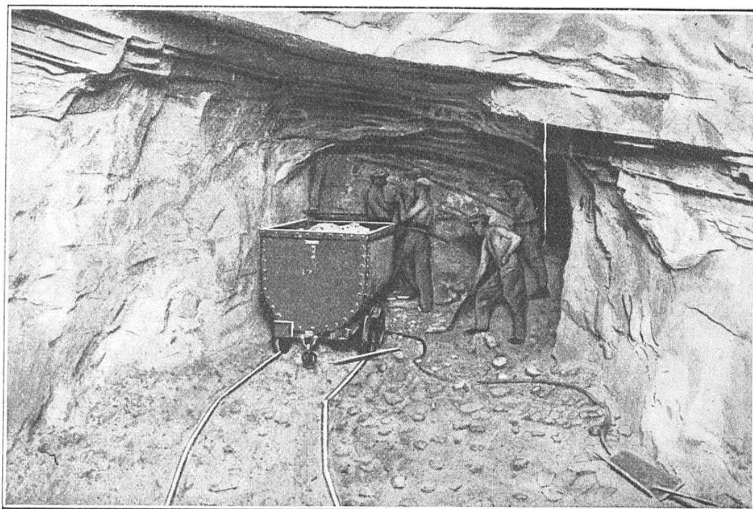
FORAGE DE TROUS DE MINES AU MOYEN DU MARTEAU PNEUMATIQUE
