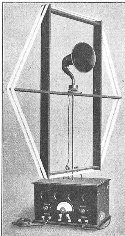
POSTE RÉCEPTEUR DE TÉLÉPHONIE SANS FIL AVEC CADRE HEXAGONAL
