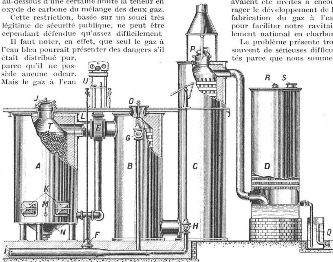
VUE EN ÉLEVATION D'UNE INSTALLATION DE GAZ A L'EAU CARBURÉ
