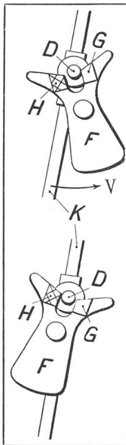
SCHÉMA DE LA FOURCHETTE PIVOTANTE DANS SES DEUX POSITIONS EXTRÊMES
