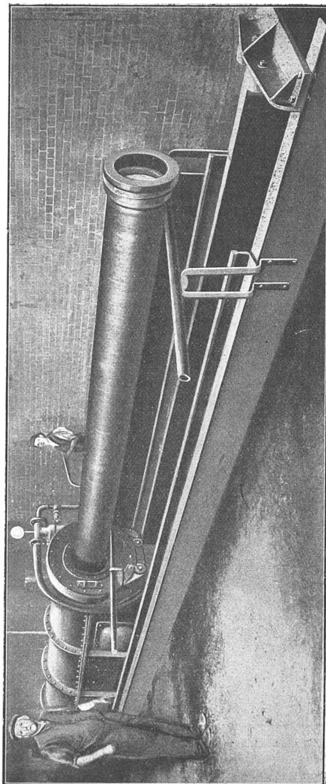
FIG. 12. — TUYAU DE FONTE DE GRANDES DIMENSIONS TEL QU'IL APPARAÎT IMMÉDIATEMENT APRÈS SA SORTIE DU MOULE Le tuyau est sorti du moule rotatif aussitôt que la fonte est prise, c'est-à-dire lorsqu'elle est à une température voisine de 800 degrés.
