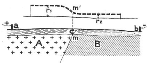
FIG. 11. — CONTACT DE DEUX TERRAINS DE CONDUCTIBILITÉS DIFFÉRENTES SOUS UNE FAIBLE ÉPAISSEUR D'ALLUVIONS HORIZONTALES. Malgré le masque d'alluvions C', qui atténue les phénomènes sans les supprimer, on peut, sur le profil de résistivités, constater facilement la résistivité plus grande du granit A (à gauche) et celle, plus faible, des schistes décomposés B (à droite).
