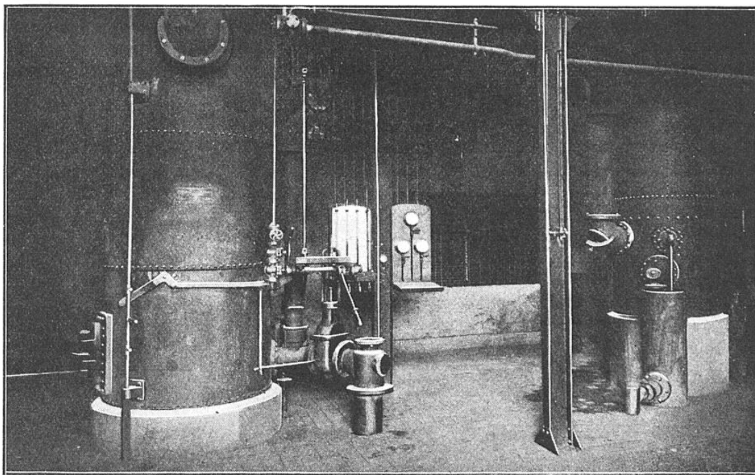
PETITE INSTALLATION DE GAZ A L'EAU BLEU, PROCÉDÉ HUMPHREYS & GLASGOW
