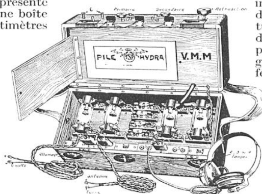
LE « PHONOBLOC » OUVERT
