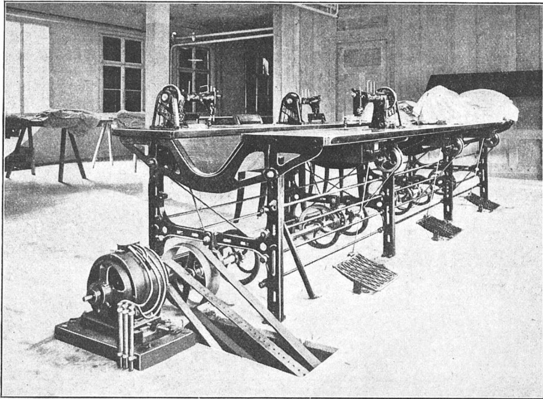
AUTRE BANC DE COUSO-MOTEURS ACTIONNÉS ÉLECTRIQUEMENT
