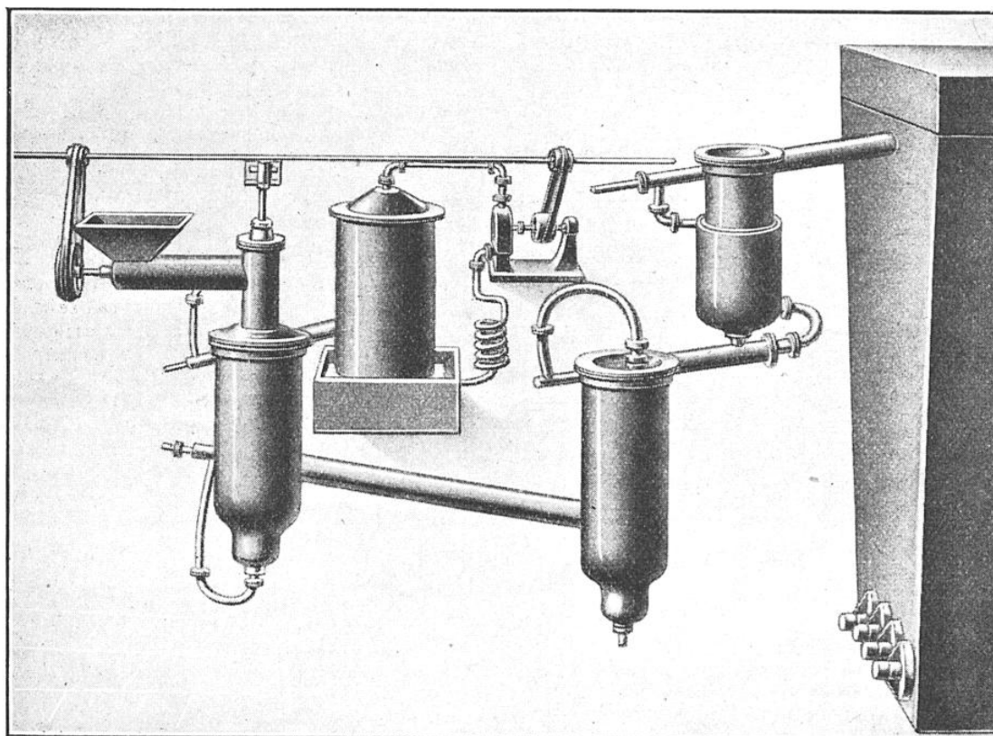
VUE D'ENSEMBLE DE L'APPAREIL AMÉRICAIN UTILISÉ POUR LA PURIFICATION RAPIDE ET ÉCONOMIQUE DU CAMPBRE NATUREL DU JAPON
