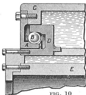
FIG. 10 ROULEMENT A BILLES REFROIDI
