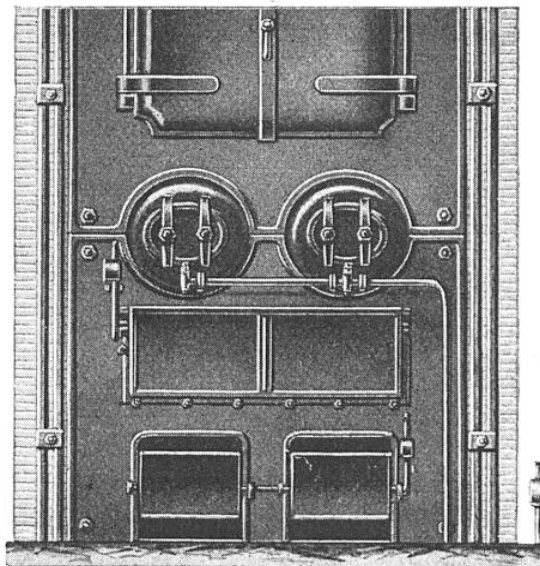
FAÇADE D'UNE CHAUDIÈRE AVEC FOYER MUNI D'UNE GRILLE POILLON, A LAMES DE PERSIENNES, AVEC SOUFFLERIE D'AIR OU DE VAPEUR
