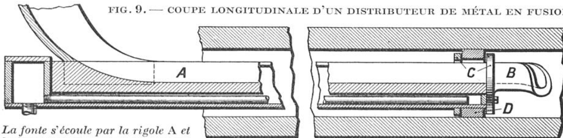
FIG. 9. — COUPE LONGITUDINALE D'UN DISTRIBUTEUR DE MÉTAL EN FUSION
