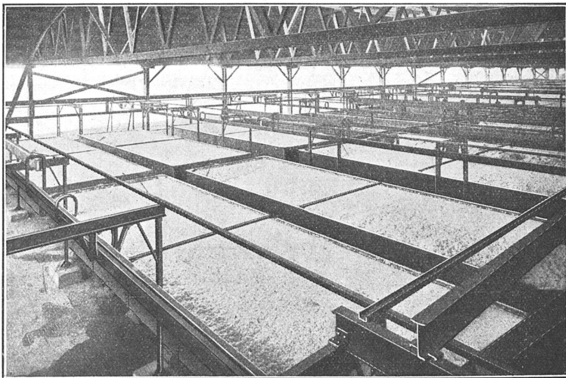
BACS DE CRISTALLISATION POUR LA FABRICATION DU CHLORURE DE POTASSIUM
