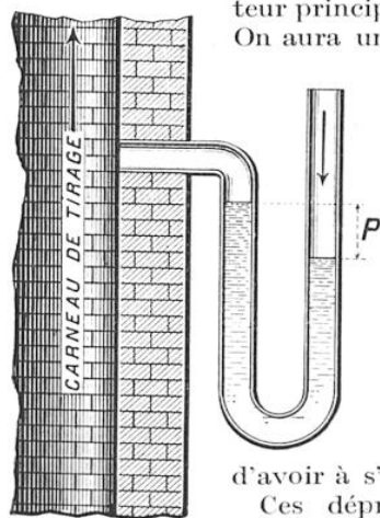
FIGURE MONTRANT LE PRINCIPE DE L'INDICATEUR HUMIDE DE TIRAGE, OU MANOMÈTRE A EAU
