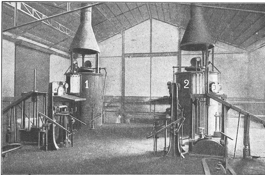
PLANCHER DE SERVICE D'UNE INSTALLATION POUR LA PRODUCTION DU GAZ A L'EAU CARBURÉ
