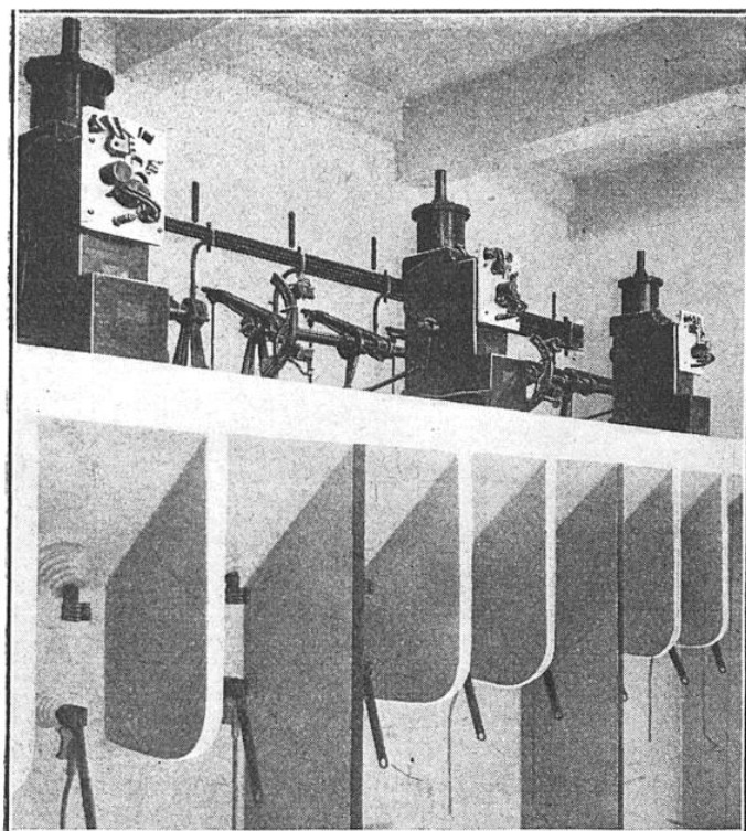
FIG. 6. — INTERRUPTEURS DE COMMANDE A DISTANCE SUR DES LIGNES A HAUTE TENSION
