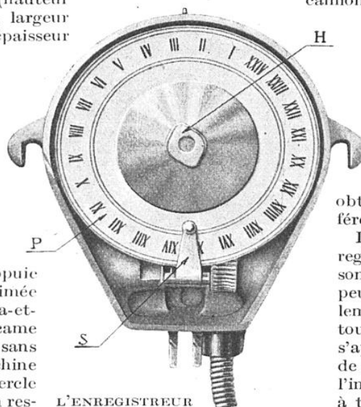
L'ENREGISTREUR AUTOMATIQUE, LE COUVERCLE ÉTANT ENLEVÉ
