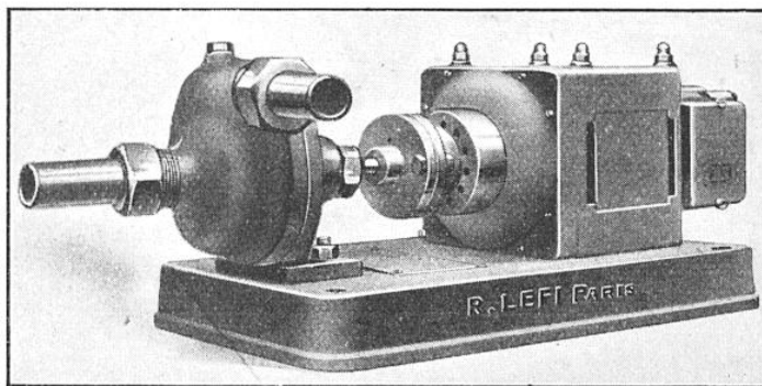
VUE D'ENSEMBLE DE LA MICROPOMPE ÉLECTRIQUE A droite, le petit moteur électrique de 1 cheval. A gauche, la turbine aspirante et foulante manœuvrée sur l'arbre du moteur.
