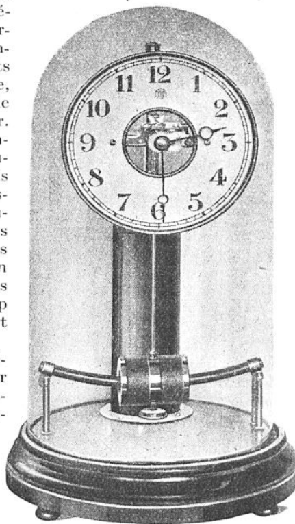
VUE D'ENSEMBLE DE L'HORLOGE ÉLECTRIQUE M. F. B.
