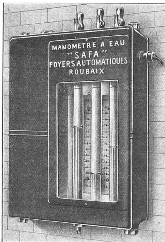
MANOMETRE A EAU « SAFA » POUR LE MÊME USAGE QUE L'APPAREIL PRÉCÉDENT, BASÉ SUR LE MÊME PRINCIPE, MAIS D'UNE CONSTRUCTION DIFFÉRENTE
