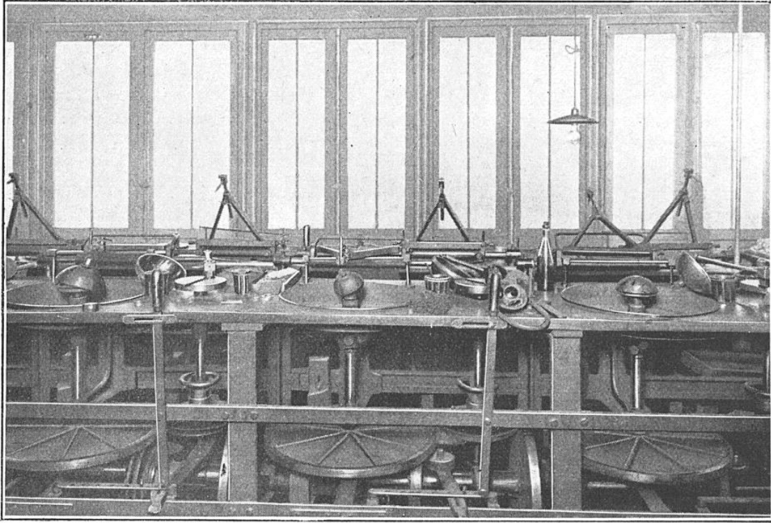
VUE PARTIELLE D'UNE MACHINE A POLIR LES LENTILLES A QUATRE PLATEAUX
