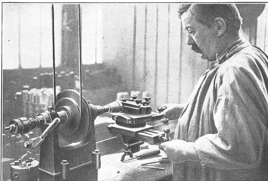
USINAGE D'UN CONE DE JUELLE SUR UN TOUR A PRISME
