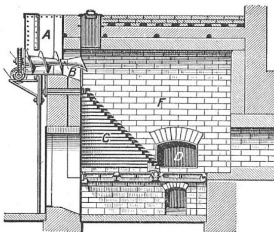
VUE EN COUPE VERTICALE D'UN FOYER POUR BRULER LES ORDURES MÉNAGÈRES
