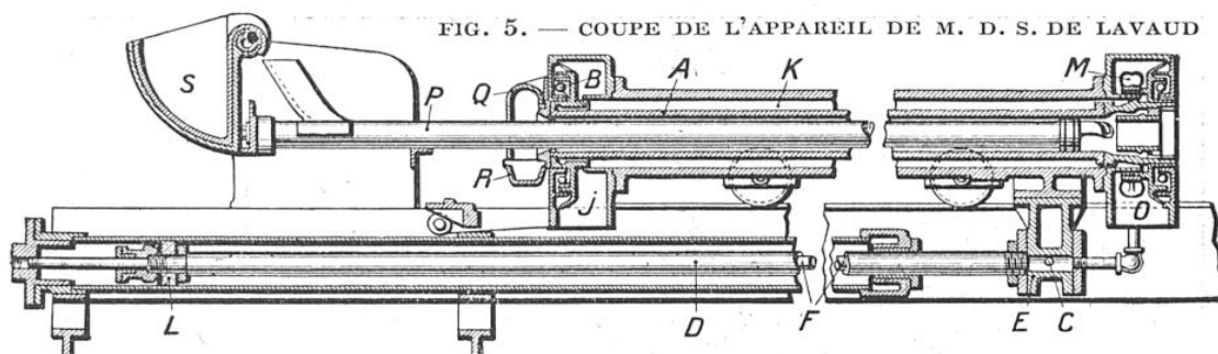
FIG. 5. — COUPE DE L'APPAREIL DE M. D. S. DE LAVAUD La fonte versée en S se rend dans le distributeur P, situé dans l'axe du moule A. Le mouvement de rotation du moule est assuré par la roue Pelton M dont l'orifice de vidange est en O. Le piston L réalise le glissement longitudinal du moule. Le support E s'ouvre dans la tige de piston D alimentée par la conduite F. L'eau passe par la conduite C et se rend ainsi dans la chemise annulaire K. Le trop-plein s'écoule par l'orifice J. Le capot Q et le bassin R empêchent le métal de s'échapper à l'extérieur du moule.
