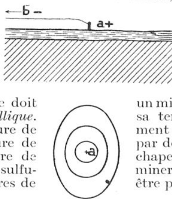
FIG. 13. — ÉTUDE D'UN TERRAIN ANISOTROPE SOUS DES MORTS-TERRAINS HORIZONTAUX
