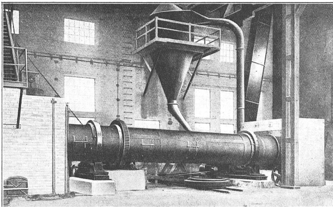
FOUR ROTATIF POUR LA DESSICCATION DU CHLORURE DE POTASSIUM
