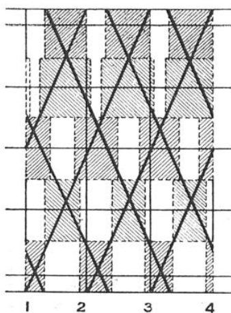
FIG. 2. - SCHÉMA MONTRANT, PAR DES SURFACES HACHURÉES, LES PÉRIODES DE FONCTIONNEMENT D'UNE SOUS-STATION DE TRACTION, POUR UN TRAIN PAR HEURE. Les parties blanches constituent l'économie de marche des machines réalisée par le système automatique.
