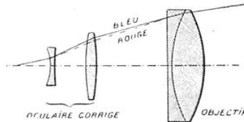
L'oculaire corrigé réduit la longueur de l'appareil et assure l'achromatisme.
