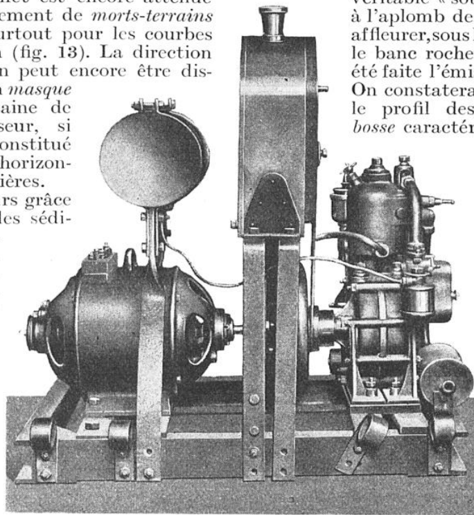
FIG. 17. — GROUPE ÉLECTROGÈNE
