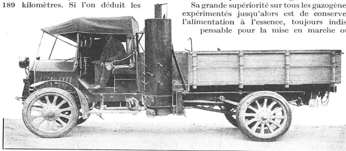
CAMION ÉQUIPÉ POUR LA MARCHÉ AU GAZ PAUVRE, AVEC GAZOGÈNE A BOIS
