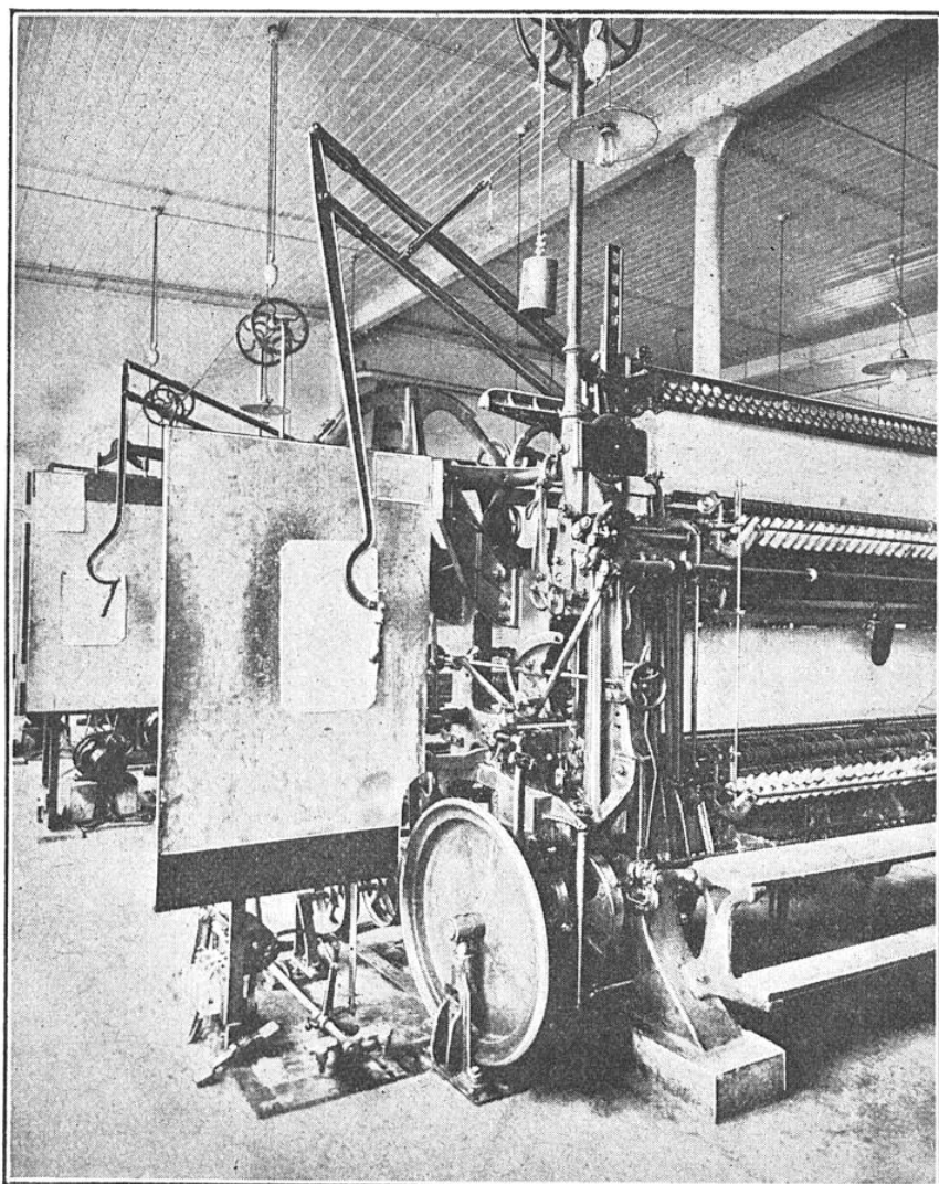
PARTIE GAUCHE DE LA FACE AVANT DU MÉTIER PLAUEEN
