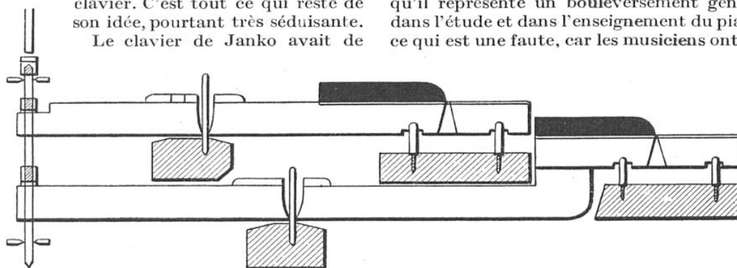
COUPE TRANSVERSALE SCHÉMATIQUE D'UN DOUBLE CLAVIER JANS
