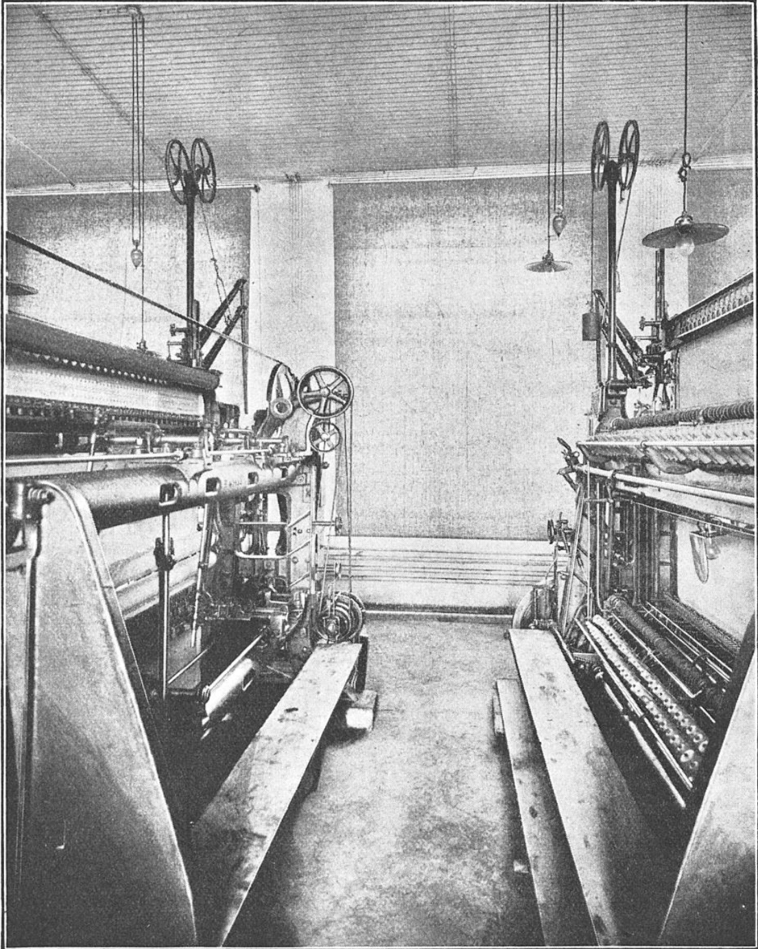
A droite : face avant du métier ; à gauche : le métier vu face arrière ; le tableau et la grande branche du pantographe pour la reproduction du dessin sont à l'arrière-plan.
