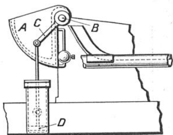
FIG. 13. — SCHÉMA DU DISPOSITIF D'ALIMENTATION DU DISTRIBUTEUR
