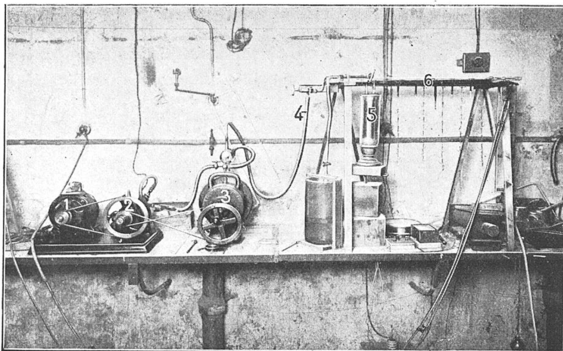
FIG. 8. — INSTALLATION DE REMPLISSAGE DES TUBES LUMINESCENTS
