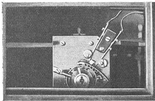
DISPOSITIF DE LA COMMANDE ÉLECTRIQUE DES SECONDES PAR L'ÉCHAPPEMENT
