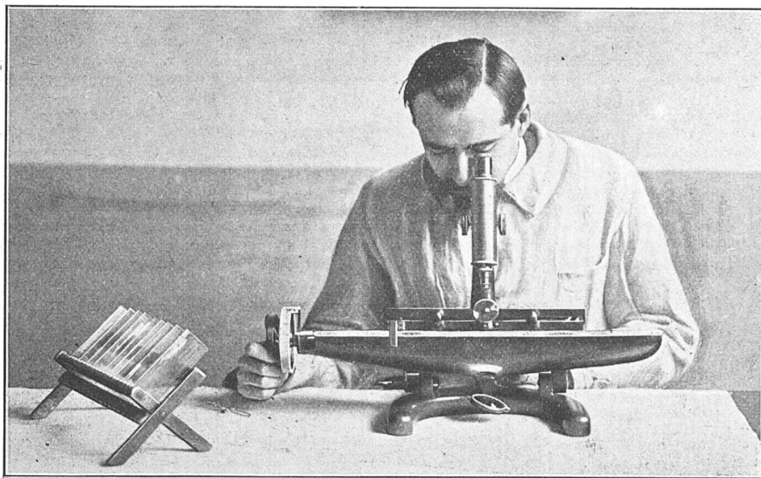
FIG. 1. — APPAREIL CONSTRUIT PAR M. BEAUDOIN POUR MESURER LES SPECTRES
