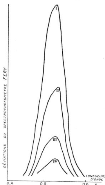
FIG. 4. — COURBE DES ABSORPTIONS SPECTRALES DE SOLUTIONS DE SAFRANINE A DIVERS ÉTATS DE DILUTION I, dilution de 12 mm. 5 par litre; II, dilution de 6 mm. 25 par litre; III, dilution de 3 mm. 125 par litre; IV, dilution de 1 mm. 56 par litre.
