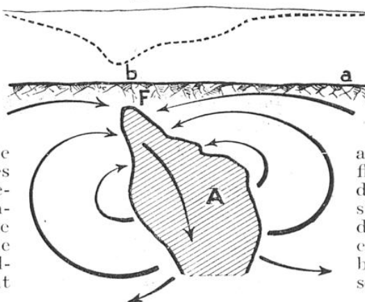
FIG. 7. — MÉCANISME DE LA « POLARISATION SPONTANÉE » D'UN GISEMENT MÉTALLIFÈRE
