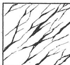
FIG. 10. — A GAUCHE : TYPE DE MINERAI ÉLECTRIQUEMENT DISCONTINU
