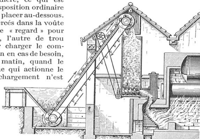
VUE D'ENSEMBLE D'UNE INSTALLATION POUR BRÛLER DES COPEAUX QUI CHAUFFENT UN GÉNÉRATEUR DE VAPEUR
