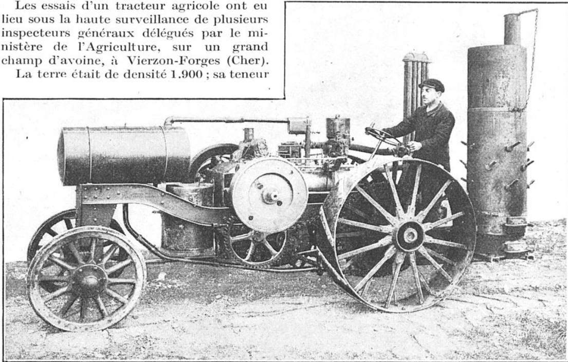
AUTRE TYPE DE TRACTEUR AGRICOLE AVEC GAZOGÈNE A GAZ PAUVRE AU BOIS
