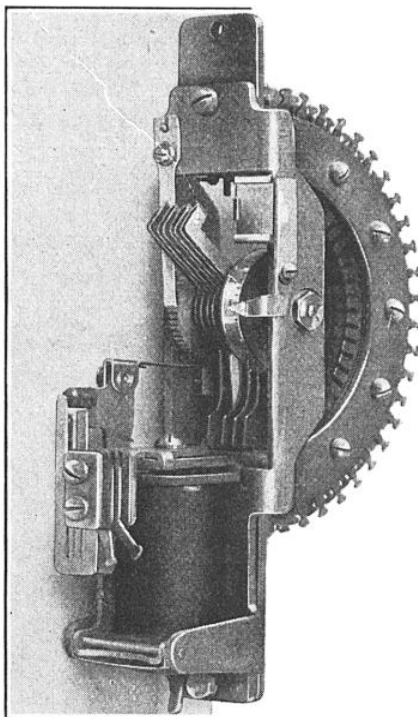
FIG. 2. — APPAREIL DISTRIBUANT AUTOMATIQUEMENT LA LIGNE DITE DE « CONVERSATION » AUX OPÉRATRICES DU BUREAU DE DÉPART.
