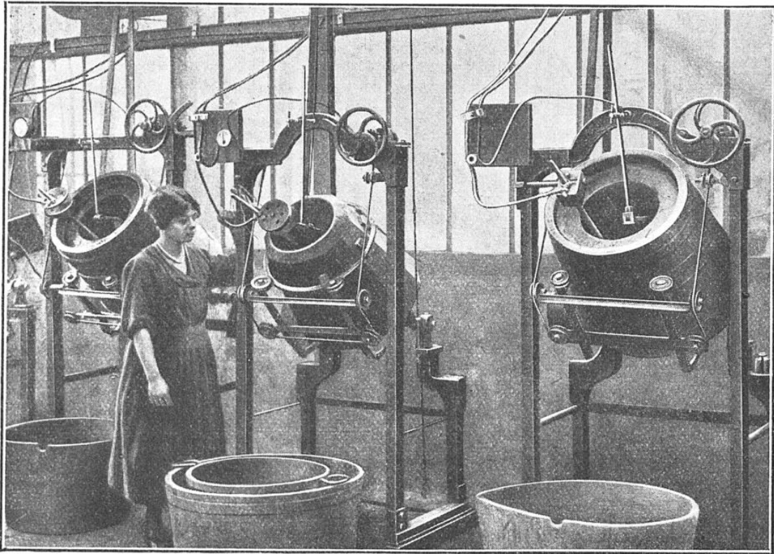
LES PIÈCES QUI NE SONT PAS ÉMAILLÉES AU FOUR SONT NICKELÉES AU TONNEAU
