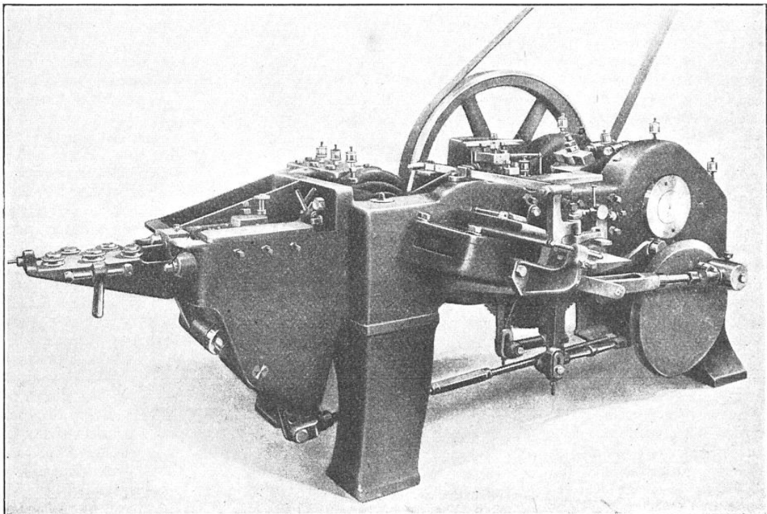
MACHINE « GALCO » POUR LA FABRICATION, EN TROIS PASSES ET A FROID, DES TÊTES DE VIS Le fil de fer ou d'acier arrive par la gauche et passe entre des galets redresseurs, puis il est coupé et saisi par des organes qui lui font subir les refolements que montre la figure de la page suivante,
