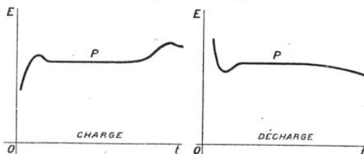
VARIATION DE LA TENSION EN FONCTION DU TEMPS PENDANT LA CHARGE ET LA DÉCHARGE D'UN ÉLÉMENT
