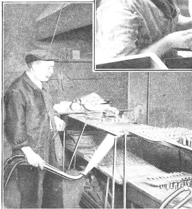
PLACÉES SUR DES GRILS MÉTALLIQUES, LES PIÈCES SONT SOUDÉES À L'AIDE DU CHALUMEAU
