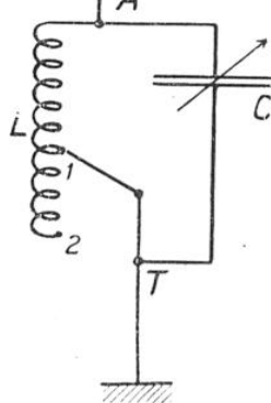
FIG. 3. — DISPOSITION DU CIRCUIT OSCILLANT POUR L'EMPLOI DU POSTE AVEC ANTENNE
