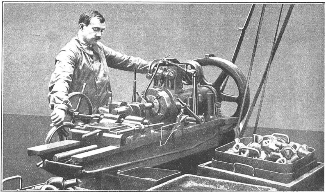
MACHINE A FILETER « ACME » DE DEUX POUCES, A VIS MÈRE
