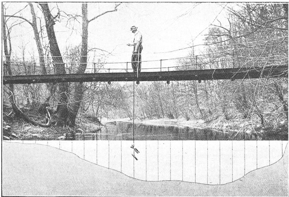
FIG. 1 — PONT FACILITANT LE JAUGEAGE D'UNE RIVIÈRE
