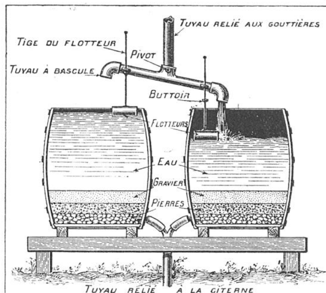
FIG. 1. — COUPE TRANSVERSALE DU SYSTÈME FILTREUR
