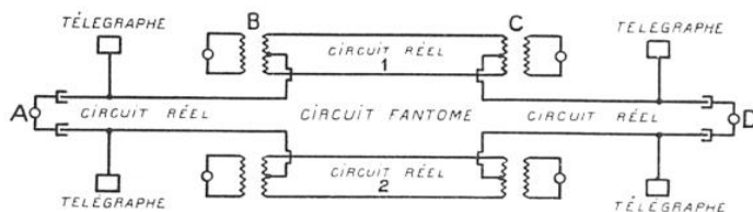
FIG. 10. — DEUX CIRCUITS RÉELS RELIENT DEUX VILLES, B ET C . ON PEUT CONSTITUER UN CIRCUIT FANTÔME QUI SERA PROLONGÉ VERS A ET D PAR DES CIRCUITS RÉELS POUR ÉTABLIR, ENTRE CES DEUX POSTES A ET D , UNE COMMUNICATION UTILISABLE POUR LE TÉLÉGRAPHE
