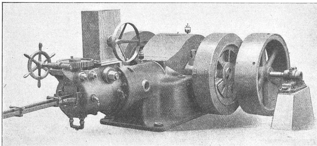
VUE DE LA MACHINE BUHLER A FABRIQUER LES BRIQUETTES DE SCIURE
