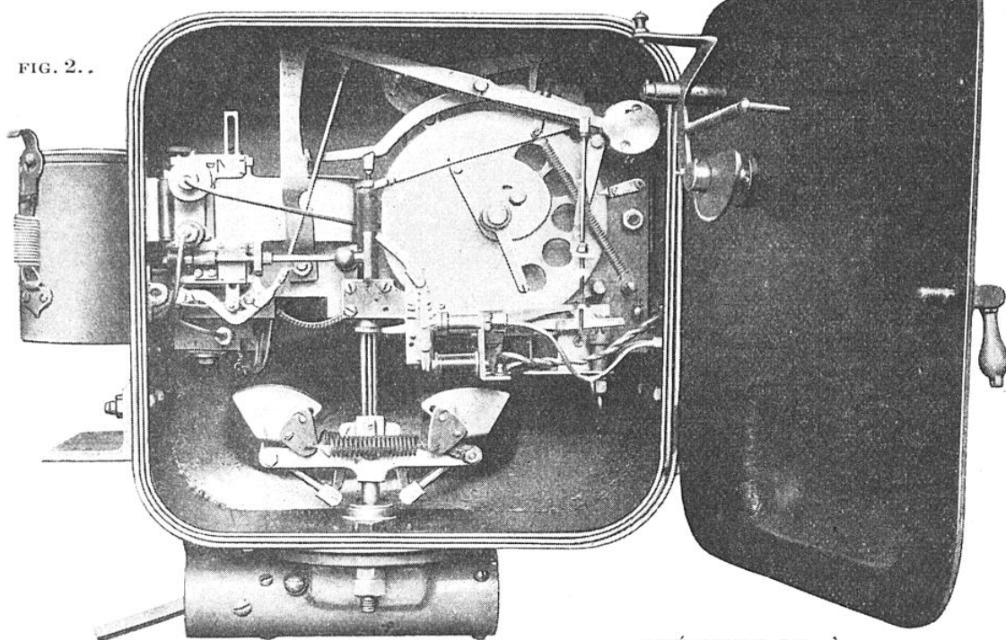
VUE INTÉRIEURE DE L'APPAREIL
