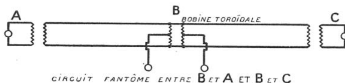
FIG. 9. — DEUX VILLES A ET C , RELIÉES PAR UN CIRCUIT RÉEL, PEUVENT ÊTRE POURVUES CHACUNE D'UNE COMMUNICATION AVEC B , EN ÉQUIPANT CE POSTE AVEC UNE BOBINE TOROÏDALE QUI DONNERA DEUX CIRCUITS FANTÔMES
