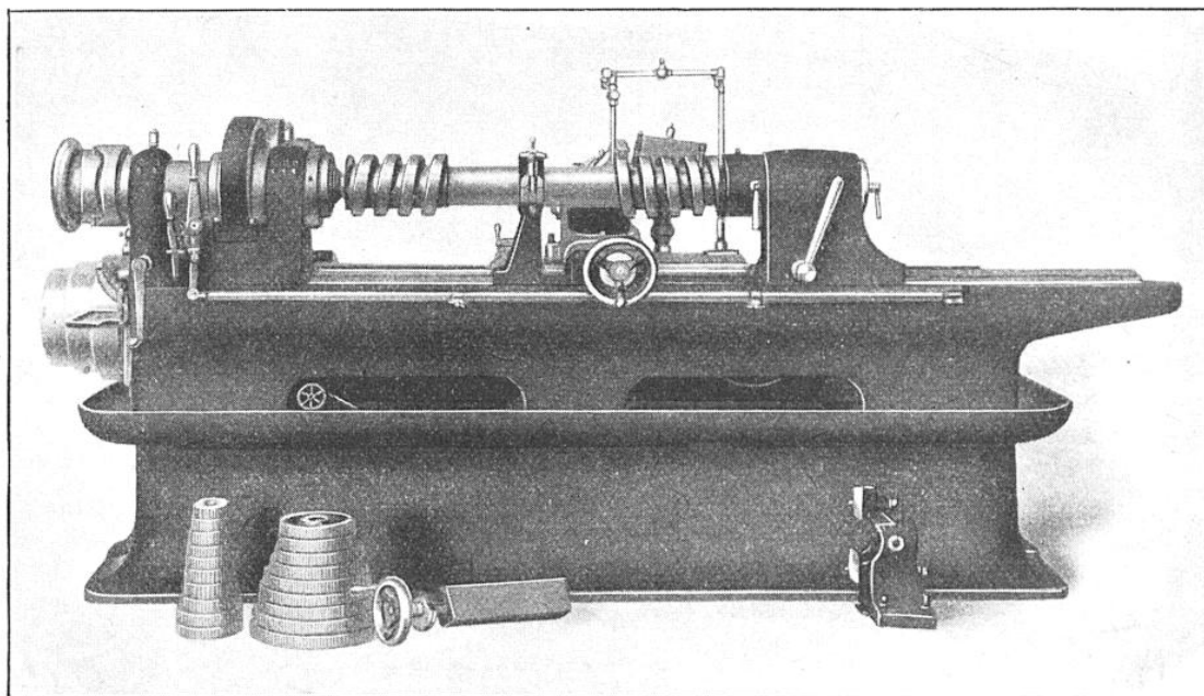
MACHINE « PRATT ET WHITNEY » POUR LE FRAISAGE DES VIS Fraisage d'une vis à filet carré, ladite vis étant montée sur une lunette fixe.
