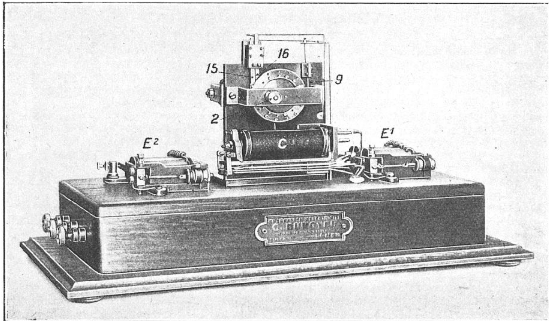
FIG. 1. — LE TÉLÉDUCTEUR DUNOIER VU DE FACE
