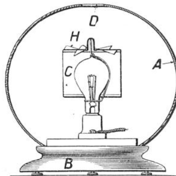
COUPE SCHEMATIQUE DU GLOBE LUMINEUX
