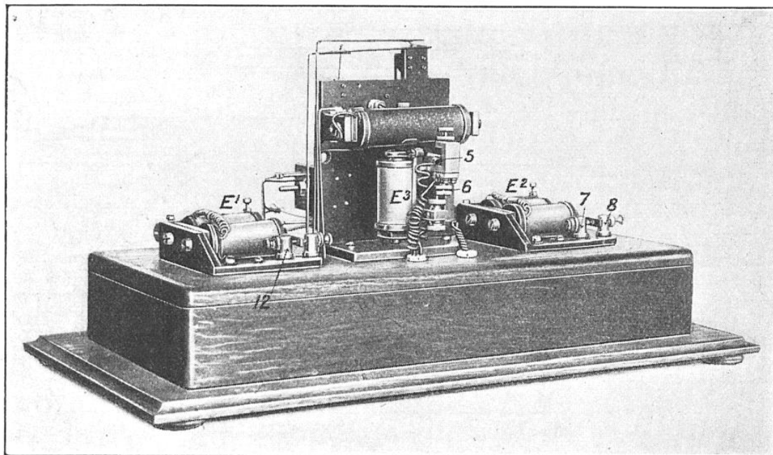
FIG. 4. — LE TÉLÉDUCTEUR DUNOYER VU PAR L'ARRIÈRE
