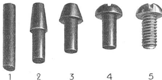
LES DIVERSES PHASES DE LA FABRICATION D'UNE VIS A MÉTAUX
