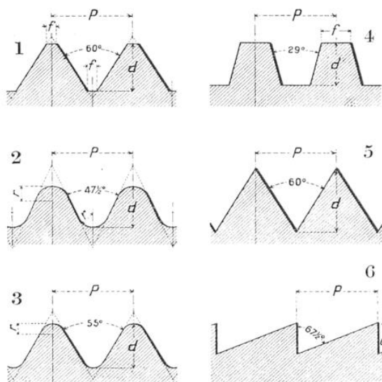
LES DIFFÉRENTS MODES DE FILETAGE DES VIS 1, système international et français, dérivé du système américain Sellers ; 2, système de la « British Association » ; 3, système Whitworth ; 4, système Acme ; 5, filets à angles vifs ; 6, clou-vis — p, pas ; d, profondeur ; f, méplat ; r, rayon.
