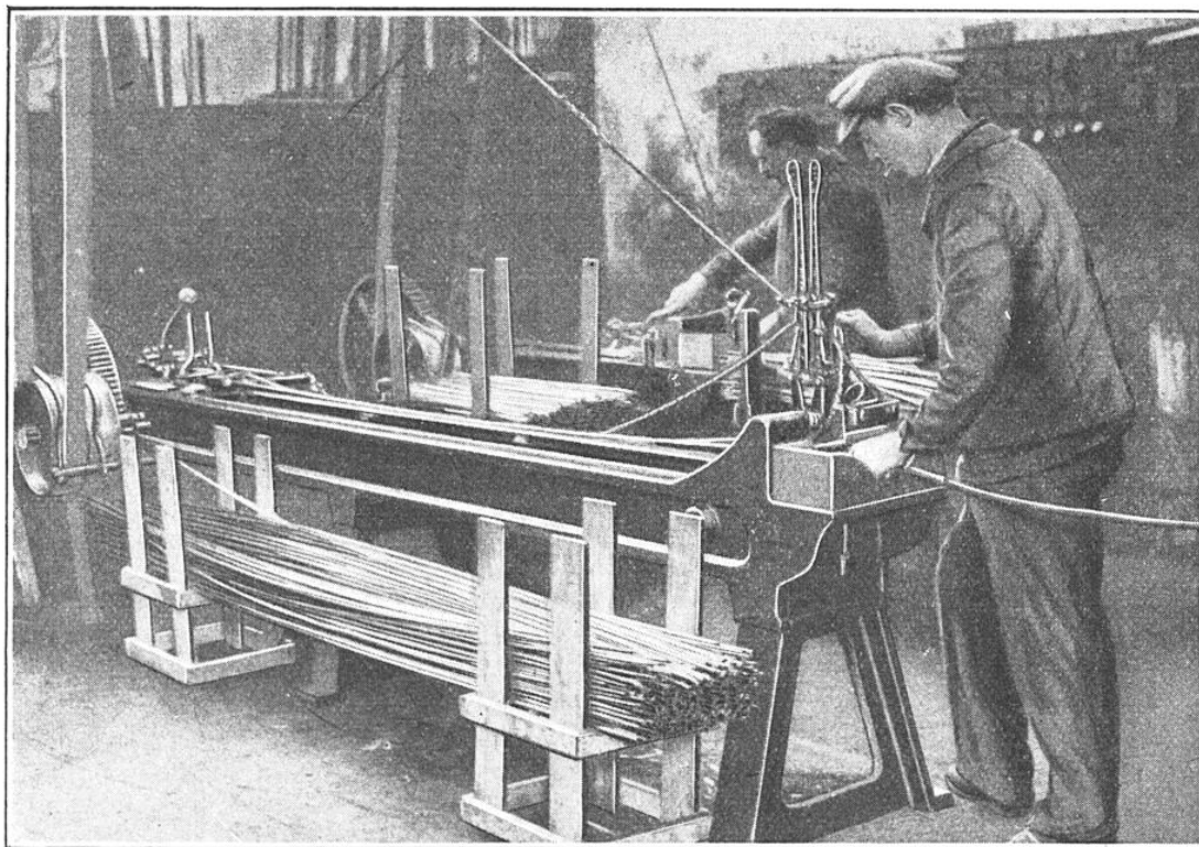
MACHINE À ÉTIRER SERVANT À FABRIQUER LES MANCHES MÉTALLIQUES DES PARAPLUIES
