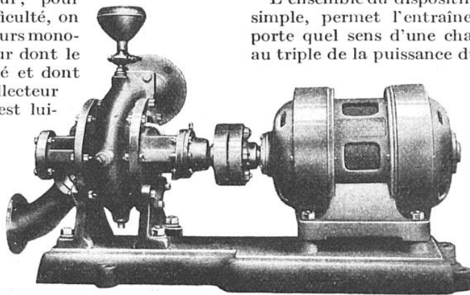
LE MOTEUR ACCOUPPLÉ AVEC UNE POMPE
