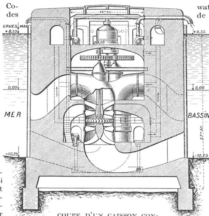
COUPE D'UN CAISSON CONTENANT DEUX TURBINES ET L'ALTERNATEUR POUR LA PRODUCTION DU COURANT
