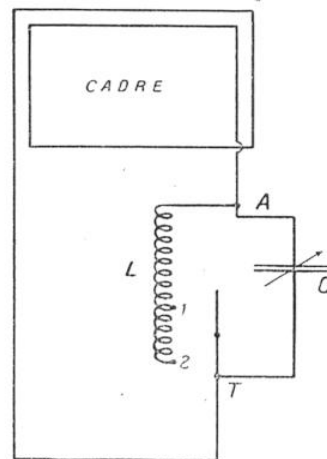
FIG. 4. — DISPOSITION DU CIRCUIT OSCILLANT POUR L'EMPLOI DU POSTE AVEC CADRE
