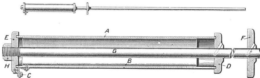
EN TOUCHANT LE CÂBLE DU CIRCUIT AVEC LA BORNE C, IL SE PRODUIT UNE PETITE ÉTINCELLE SI LE CIRCUIT EST SOUS TENSION
