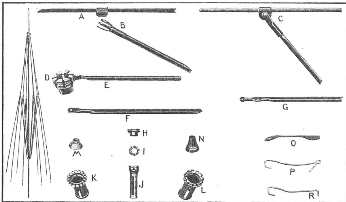
UNE CARCASSE DE PARAPLUIE COMPORTE D'ASSEZ NOMBREUSES PIÈCES
