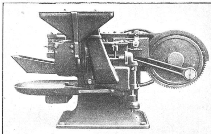
MACHINE « GALCO » A FILETER LES VIS A MÉTAUX PAR ENROULEMENT DU FUT ENTRE DES MATRICES PLANES
