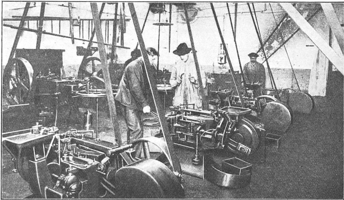
ATELIER DANS UNE GRANDE FABRIQUE DE VIS OU SONT UTILISÉES LES MACHINES « GALCO »
