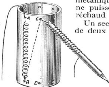
MANIÈRE DE PRÉPARER LES ÉLÉMENTS CHAUFFANTS
