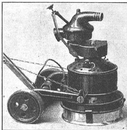
L'ASPIRATEUR SE PLACE AISÉMENT SUR LE MOTEUR DONT L'AXE EST VERTICAL
