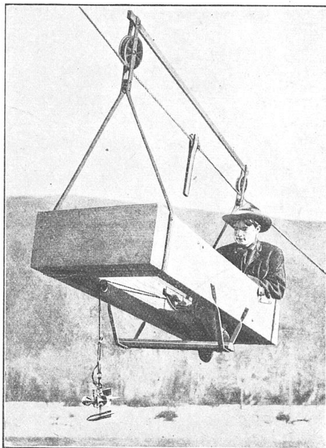
FIG. 3. — CHARIOT SOUTENU PAR UN CABLE D'ACIER AU DESSUS D'UN TORRENT OU D'UN FLEUVE AUX RIVES ESCARPÉES
