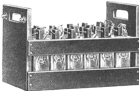
BATTERIE DE PILES FÉRY POUR T. S. F.
