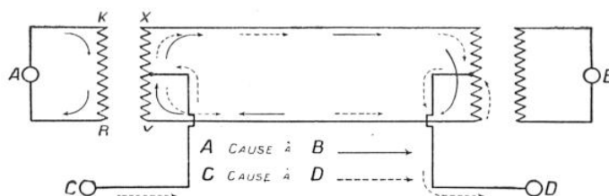
FIG. 5. — SCHÉMA DE LA MARCHÉ DES COURANTS DANS UN CIRCUIT RÉEL ET DANS UN CIRCUIT FANTÔME
