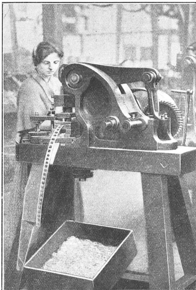
L'EMPORTE-PIÈCE ENLÈVE DANS LA TOLE DES RONDELLES, DES CARRÉS, DES ÉTOILES QUI CONSTITUERONT AUTANT DE PIÈCES DÉTACHÉES
