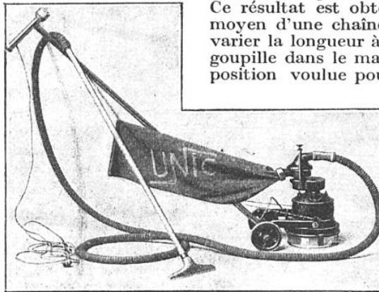
L'ÉLECTRO-CIREUSE DISPOSÉE AVEC SON ASPIRATEUR DE POUSSIÈRES
