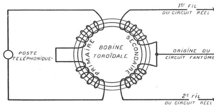
FIG. 2. — BOBINE TOROÏDALE EMPLOYÉE DANS L'ÉQUIPEMENT DES CIRCUITS RÉELS POUR RÉALISER LES CIRCUITS DÉNOMMÉS CIRCUITS FANTOMES PAR LES AMÉRICAINS
