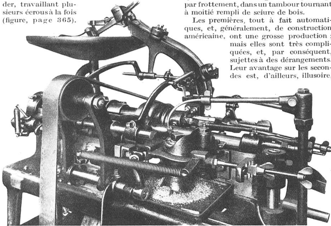
MACHINE « GALCO » POUR TOURNER ET FENDRE LES TÊTES DE VIS A BOIS
