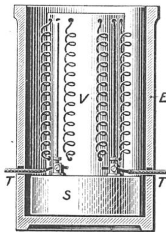
VUE INTÉRIEURE DE L'APPAREIL DE CHAUFFAGE
