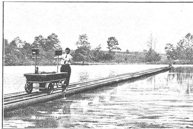
FIG. 5. — CHARIOT ROULANT SUR DES RAILS DISPOSÉS LE LONG D'UN BARRAGE ET AMENANT LES APPAREILS HYDRAULIQUES A PIED D'ŒUVRE
