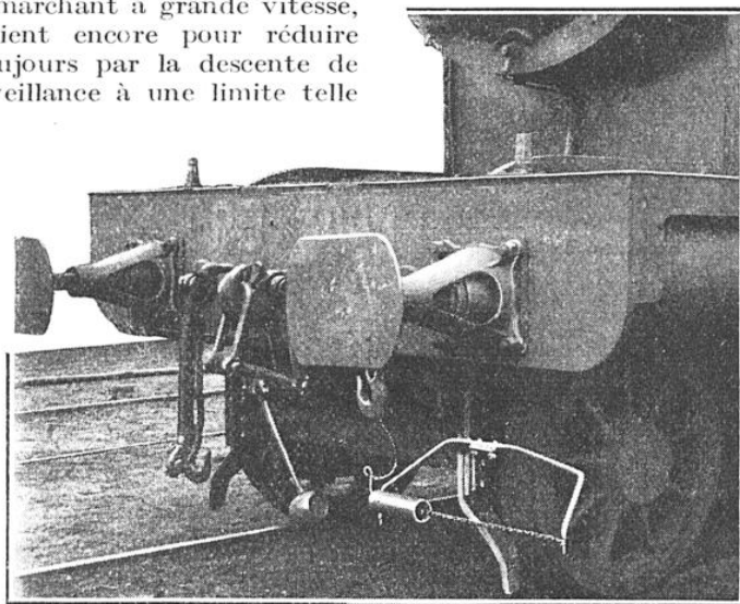
FIG. 6. — L'APPAREIL RÉCEPTEUR
