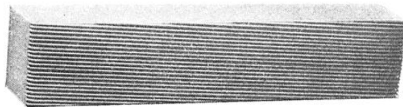
MATRICE PLANE, OU PLATEAU-FILIÈRE, EN ACIER TREMPÉ, UTILISÉE DANS LA MACHINE PRÉCÉDENTE Cette matrice porte en creux le développement rectiligne du filetage hélicoïdal.
