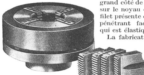
FILIÈRE AJUSTABLE MODÈLE « GRANT »
