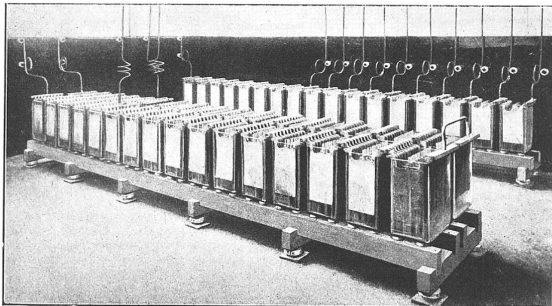
VUE D'ENSEMBLE D'UNE BATTERIE STATIONNAIRE OU BATTERIE-TAMPON
