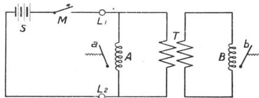
FIG. 2. — PRINCIPE DE L'APPAREIL TÉLÉDUCTEUR
