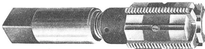
TARAUD EXPANSIBLE « PRATT ET WHITNEY » POUR LE PAS WHITWORTH
