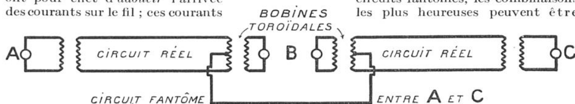
FIG. 8. — CONSTITUTION D'UN CIRCUIT FANTÔME ENTRE A ET C À L'AIDE DES CIRCUITS RÉELS AB ET BC ÉQUIPÉS AVEC DES BOBINES TOROÏDALES AU POSTE B
