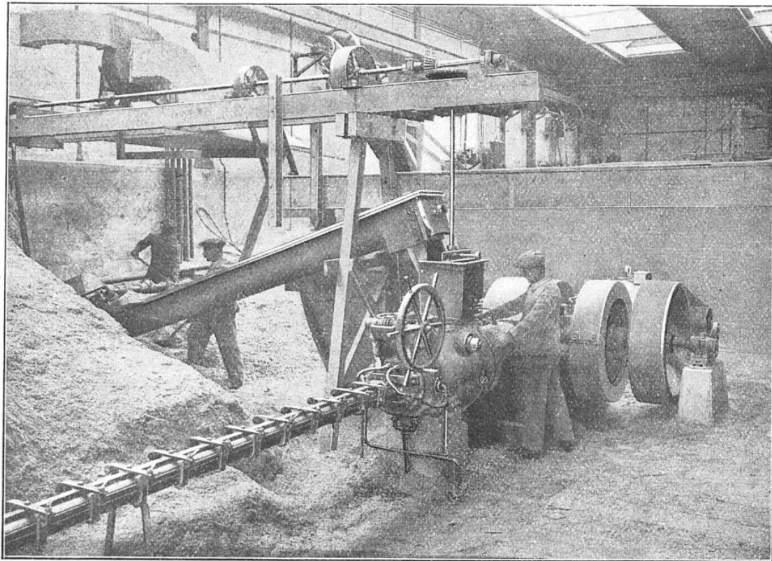
LA MACHINE A BRIQUETTES DE SCIURE EN PLEIN FONCTIONNEMENT
