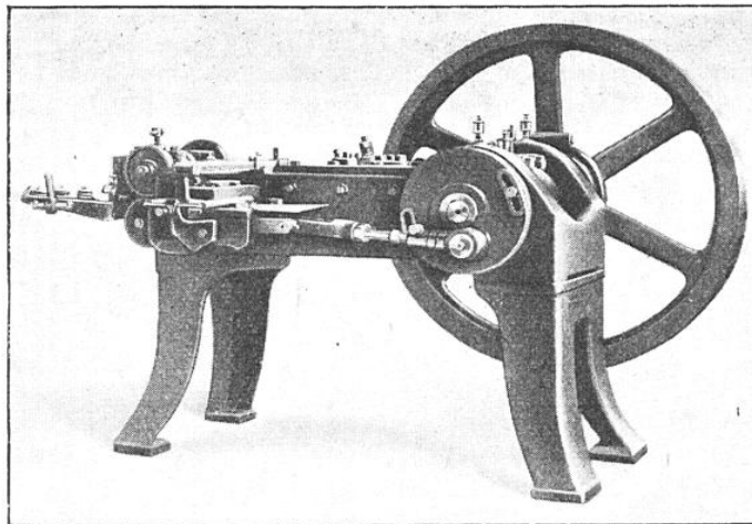
MACHINE « GALCO » POUR FABRIQUER, PAR REFOULEMENT A FROID, EN UNE SEULE PASSE, LES TÊTES DE RIVETS DE FAIBLE DIAMÈTRE
