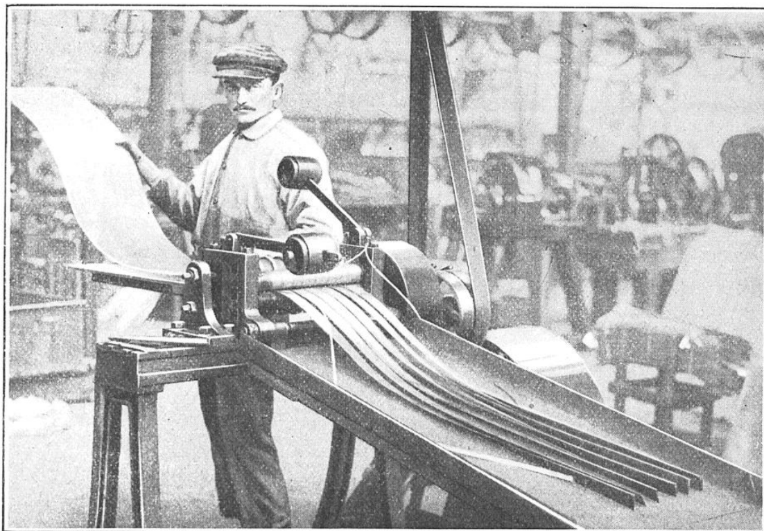
DÉCOUPAGE DES PLAQUES DE TOLE POUR FABRIQUER LES NOIX ET LES COULISSEUX
