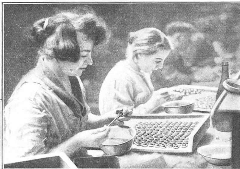
LES NOIX ET LES COULISSEUX SONT PASSÉS AU CUIVRE ET AU BORAX POUR FACILITER LA SOUDURE DES PIÈCES QUI LES COMPOSENT
