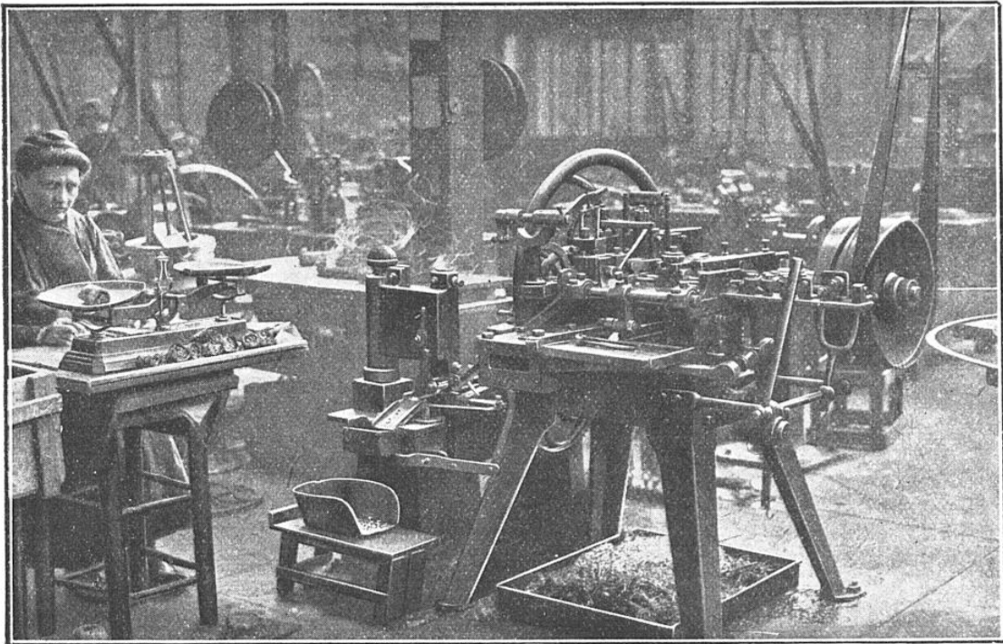
MACHINE A FAIRE LES RESSORTS QUE L'ON VOIT A LA PAGE 377, EN « P » ET « R » Le fil d'acier est plié, tordu, mis à la forme et débité par grosses.
