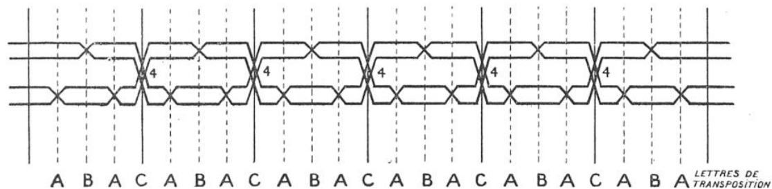
FIG. 4. — TRANSPOSITION DES FILS ET DES CIRCUITS TÉLÉPHONIQUES POUR PERMETTRE L'ÉQUIPEMENT D'UN CIRCUIT FANTÔME
