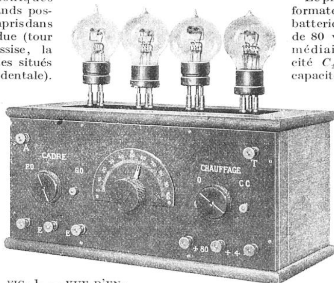
FIG. 1. — VUE D'ENSEMBLE D'UN POSTE A QUATRE LAMPES « INNOVATION »
