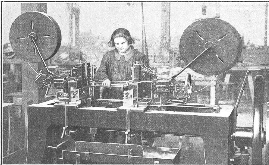
FAÇONNAGE AUTOMATIQUE DES EXTRÉMITÉS DES BRANCHES MÉTALLIQUES DES PARAPLUIES Des chaînes de Galle présentent les branches devant une série d'outils qui les achèvent.
