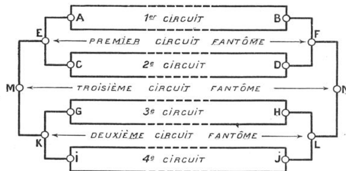
FIG. 1. — QUATRE CIRCUITS RÉELS PERMETTANT LA FORMATION DE TROIS CIRCUITS FANTOMES AB, CD, GH, IJ, circuits réels ; EF, KL, MN, circuits fantômes.
