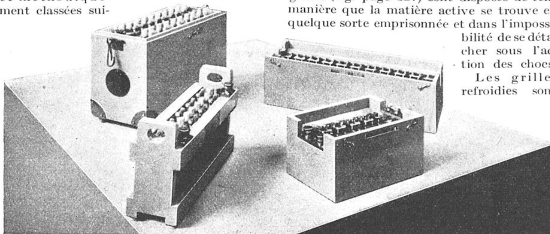
QUELQUES AUTRES TYPES DE BATTERIES D'ACCUMULATEURS POUR T. S. F.
