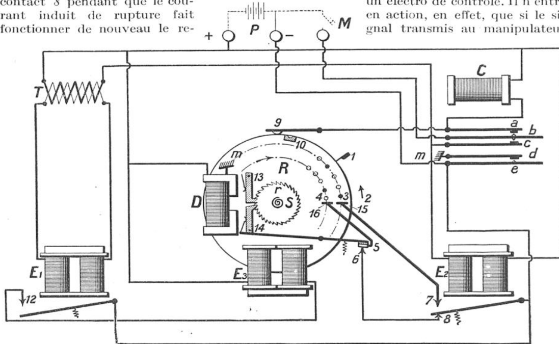
FIG. 3. — SCHÉMA D'ENSEMBLE DU TÉLÉDUCTEUR DUNOYER
