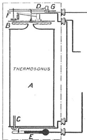
COUPE DE L'APPAREIL
