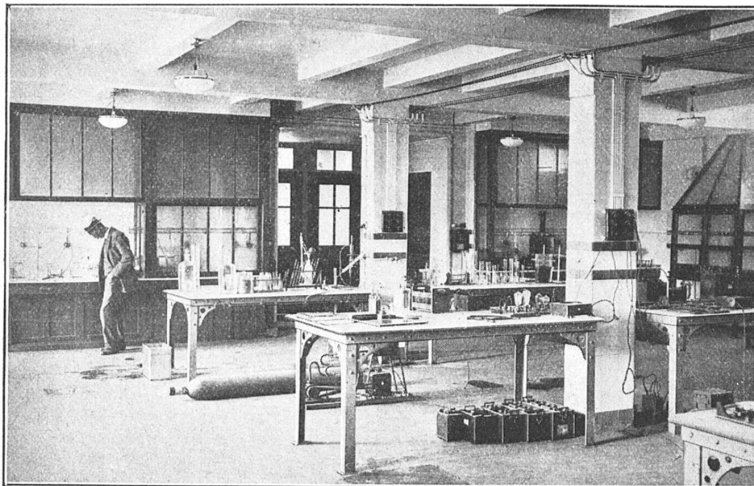
LABORATOIRE DE VÉRIFICATION DANS UNE FABRIQUE D'ACCUMULATEURS
