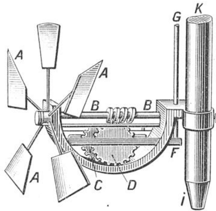
FIG. 4. — MOULINET DE WOLTMANN A , ailettes ; B B , arbre ; F G , tringle verticale ; C D , roues dentées ; K I , tige.
