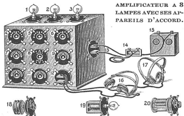
L'appareil est entièrement monté avec des éléments « Omnibus ». On remarque sur la figure : un disque avec dispositif de réation (18), douilles d'audion et transformateur (19), condensateur variable (20), et casques avec écouteurs (16 et 17).
