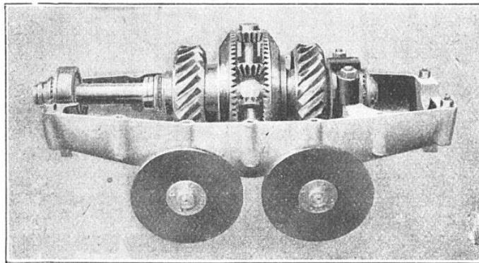
LE PONT ARRIÈRE DU CHASSIS DESMOULIN
