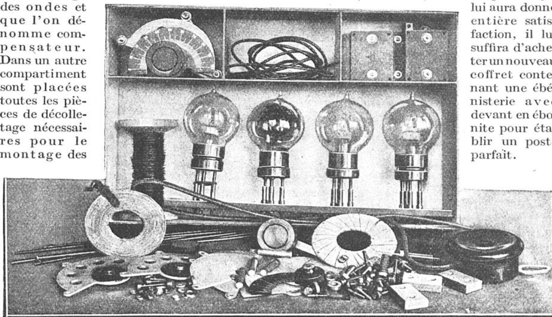
VUE DU « RADIO-BOX » OUVERT ET DES NOMBREUSES PIÈCES DE MONTAGE QU'IL CONTIENT
