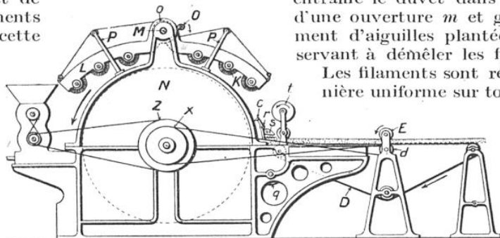
VUE EN ÉLÉVATION D'UNE CARTE A KAPOK
