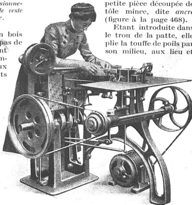
MACHINE LAILE, DU SYSTÈME A ANCRE, A MOTEUR ÉLECTRIQUE, DONNANT SENSIBLEMENT LA MÊME PRODUCTION QUE LA PRÉCÉDENTE
