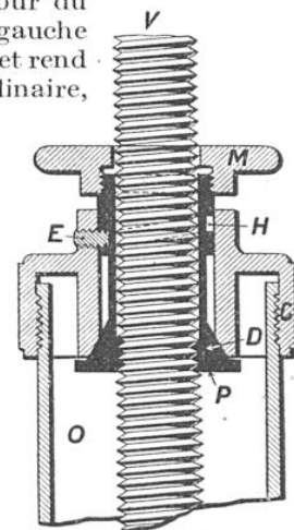
COUPE DU CHAPEAU DE LA POMPE
