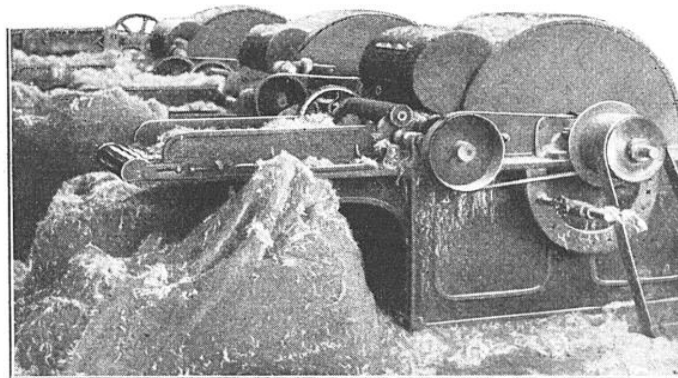
MACHINE A NETTOYER ET A ÉGRENER LE KAPOK
