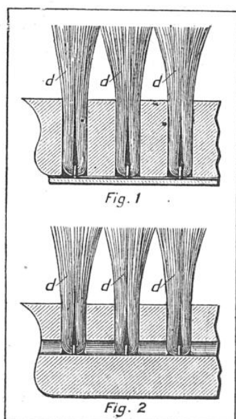
DEUX PROCÉDÉS DE MONTAGE Fig. 1 : Montage d'un bois percé de part en part ; d, touffe du loquet faisant saillie au dehors. — Fig. 2 : Montage d'un bois percé seulement sur une partie de son épaisseur, avec canal longitudinal où viennent aboutir les fonds des trous.
