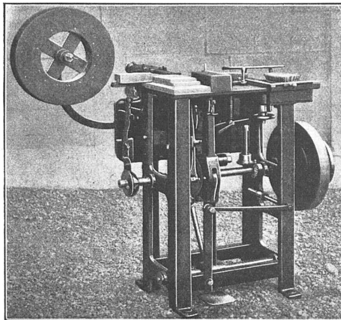
MACHINE DU SYSTÈME A BOUCLE, FONCTIONNANT A LA PÉDALE, POUR PETITE PRODUCTION
