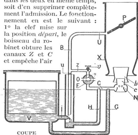
DU CARBURATEUR A TRIPLE DIFFUSEUR
