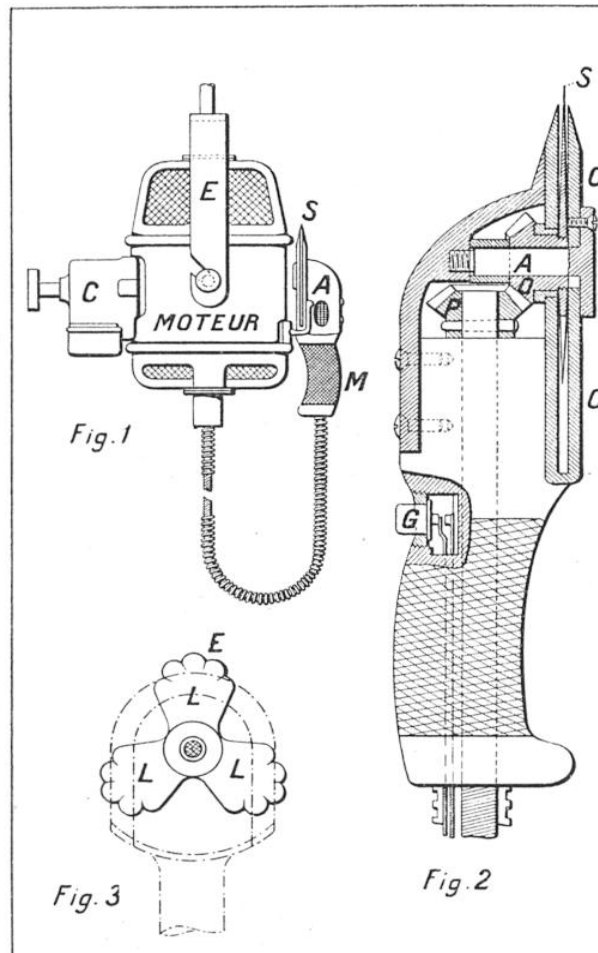
FIG. 2. — DÉTAILS DE CONSTRUCTION DU « PERCO » 1. Le Perco suspendu à son moteur électrique. M , poignée ; A , monture ; S , outil séparateur ; C , commutateur ; E , étrier de suspension du moteur. — 2. P O , pignons dentés transmettant le mouvement à l'arbre A porteur de l'outil S ; C , carter de l'outil ; G , commutateur. — 3. L L , outil séparateur à trois branches ; E , parties de l'outil agissant comme des marteaux pour détacher la peau de l'animal.
