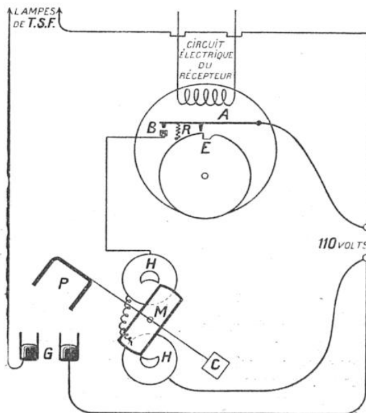
FIG. 8. — SCHÉMA DU RELAIS A MERCURE
