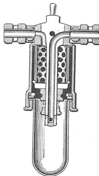
COUPE DU FILTRE DE PRÉCISION
