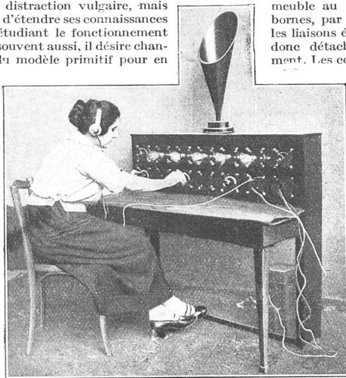
RADIO-TABLE PLIANTE A CINQ LAMPES
