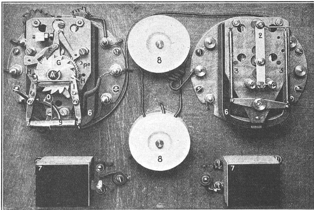
FIG. 6. — LE RELAIS SENSIBLE ET LE RELAIS RETARDÉ
