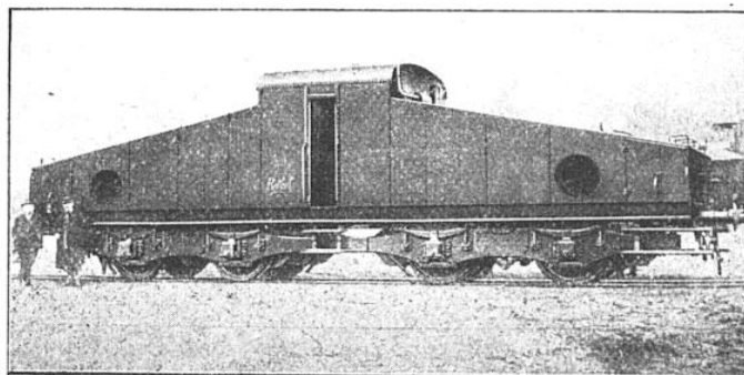
FIG. 7. — LOCOMOTIVE A ESSENCE ET A TRANSMISSION ÉLECTRIQUE HENRY CROCHAT, POUR VOIES NORMALES
