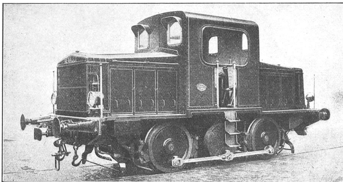
FIG. 1. — LOCOMOTIVE A ESSENCE RENAULT, DE 60 CHEVAUX, POUR VOIES FERRÉES
