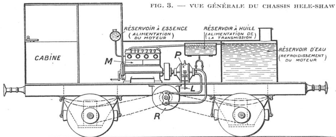
M. moteur à essence actionnant la pompe P ; L, levier de commande de la pompe ; R, moteur récepteur actionné par la pompe et transmettant sa puissance aux roues motrices par l'intermédiaire de chaînes.
