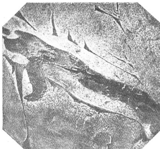
COMPARAISON DE LA STRUCTURE DU FER DE CAILLE (FIG. SUPÉRIEURE) AVEC CELLE DU FER DE CANYON-DIABLO
