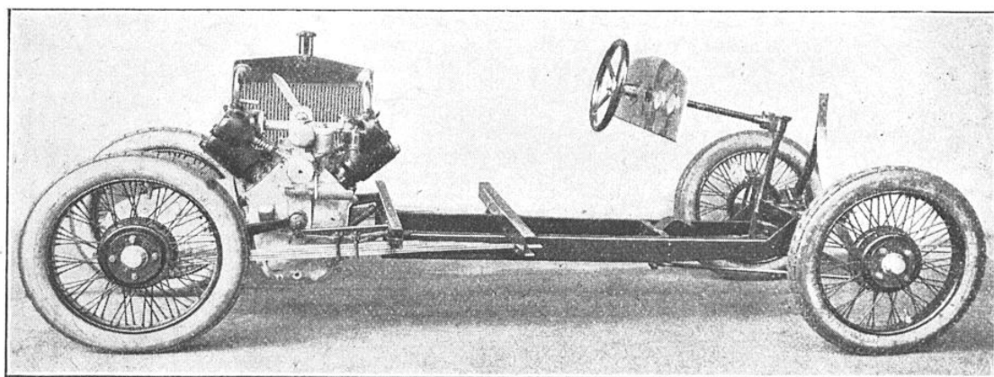
CHASSIS PARTICULIÈREMENT ORIGINAL DE LA VOITURE JANEMIAN
