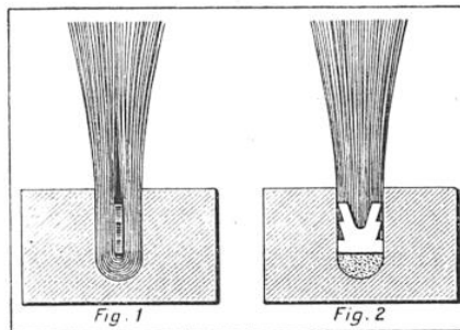
PROCÉDÉ DE MONTAGE DE M. DE MONT Dans ce système, le fil de ligature est remplacé par une petite pièce en tôle mince dite « ancre » enfoncée avec le loquet par un poinçon. — Fig. 1 : vue de profil de l'ancre ; fig. 2 : vue de face de l'ancre, le loquet étant supposé coupé dans sa partie repliée.
