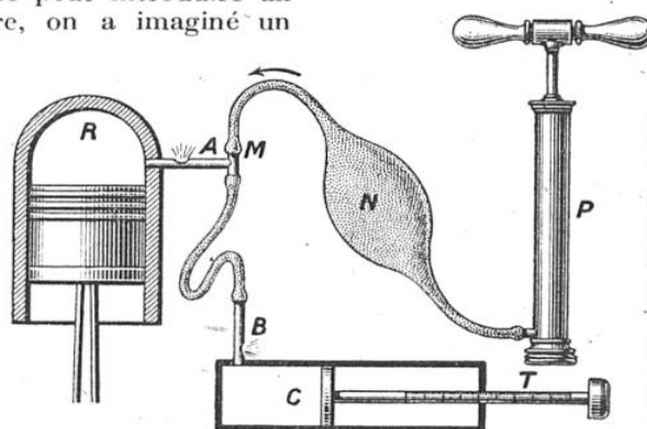
SCHÉMA DU VOLUMÈTRE ACOUSTIQUE
