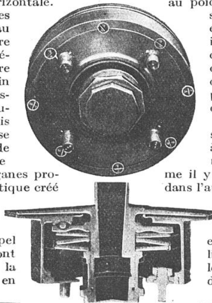
LE « FREIN DE CENTRE » (VUE EXTÉRIEURE ET COUPE)
