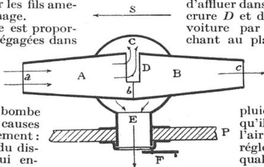
COUPE DU SOUFFLEUR CHANARD
