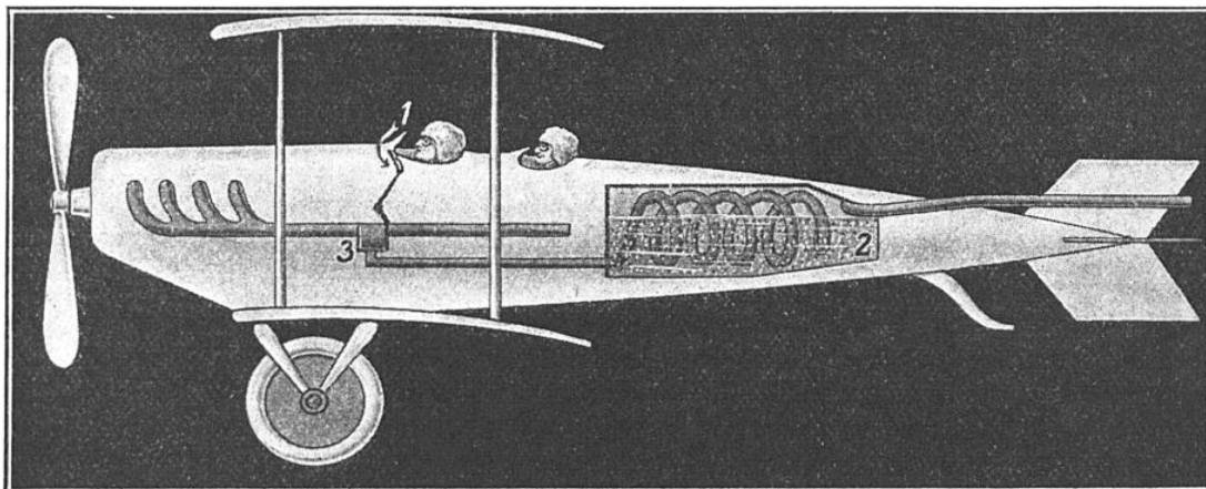
1, levier de contrôle des émissions de fumée ; 2, réservoir métallique contenant les huiles et les produits chimiques servant à produire la fumée ; 3, soupape servant à refouler les gaz d'échappement du moteur à travers le tube et le serpentín perforé plongeant dans le liquide producteur de fumée.
