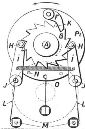
FIG. 5. — VUE DE FACE DU MÉCANISME DE RELAIS RETARDÉ (VOIR FIG. 4)
