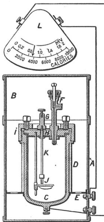
COUPE DE LA BOMBE CALORIMÉTRIQUE FÉRY
