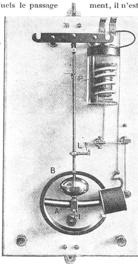
MÉCANISME INTÉRIEUR DE LA PENDULE « HÉLIOS »
