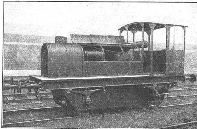
FIG. 5. — LOCOTRACTEUR PÉTROLÉO-HYDRAULIQUE HELE-SHAW DE 20 CHEVAUX ET DU POIDS DE 9 TONNES
