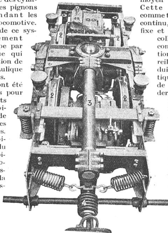
FIG. 6. — BOGIE, VU PAR-DESSUS, D'UN LOCOMOTRACTEUR HENRY CROCHAT POUR VOIE DE 60 CENTIMÈTRES DE LARGEUR
