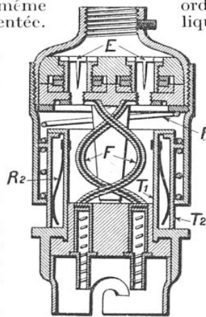
COUPE DU PORTE-LAMPES AMORTISSEUR
