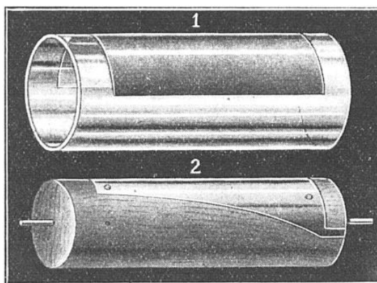
DÉTAILS DU CONDENSATEUR RÉGLABLE : 1, verre de lampe sur lequel on a collé une bande d'étain ; 2, armature interne constituée par un cylindre de bois portant également une feuille d'étain.
