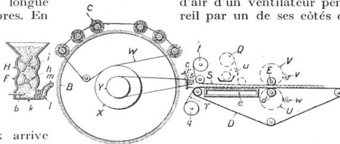
COUPE VERTICALE SCHÉMATIQUE D'UNE MACHINE A CARDER LE KAPOK
