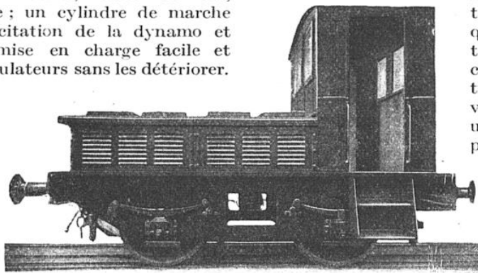
FIG. 8. — LOCOMOTIVE ÉLECTRIQUE A ACCUMULATEURS HENRY CROCHAT POUR VOIES NORMALES (12 TONNES)
