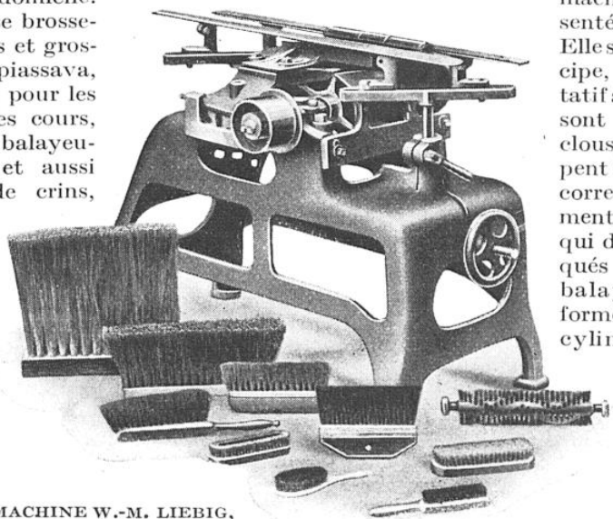
MACHINE W.-M. LIEBIG, PERMETTANT DE TONDRE (OU COUPER LE RANG) LES BROSSES DE TOUTES DIMENSIONS, ET MÊME LES BROSSES CYLINDRIQUES
