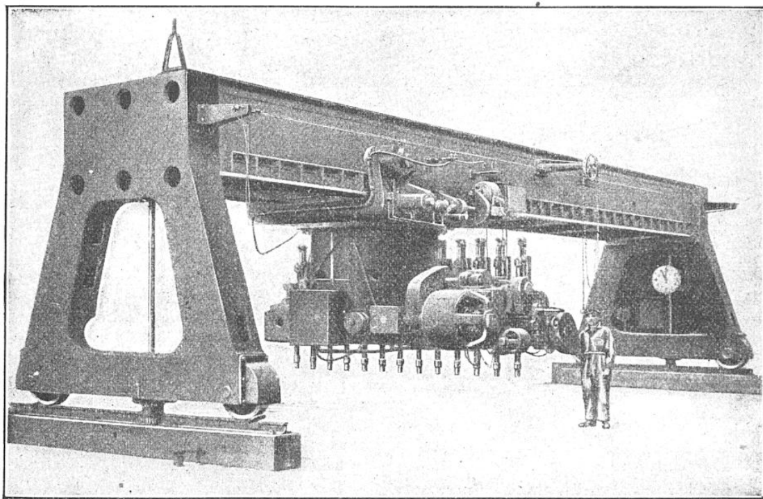
PONT ROULANT SUPPORTANT LA PERCEUSE A TREIZE FORETS
