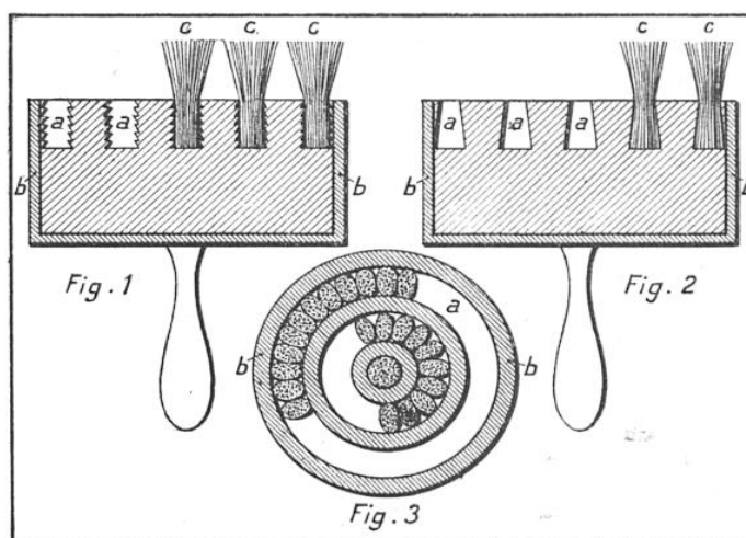
PROCÉDÉ DE MONTAGE SYSTÈME MASON
