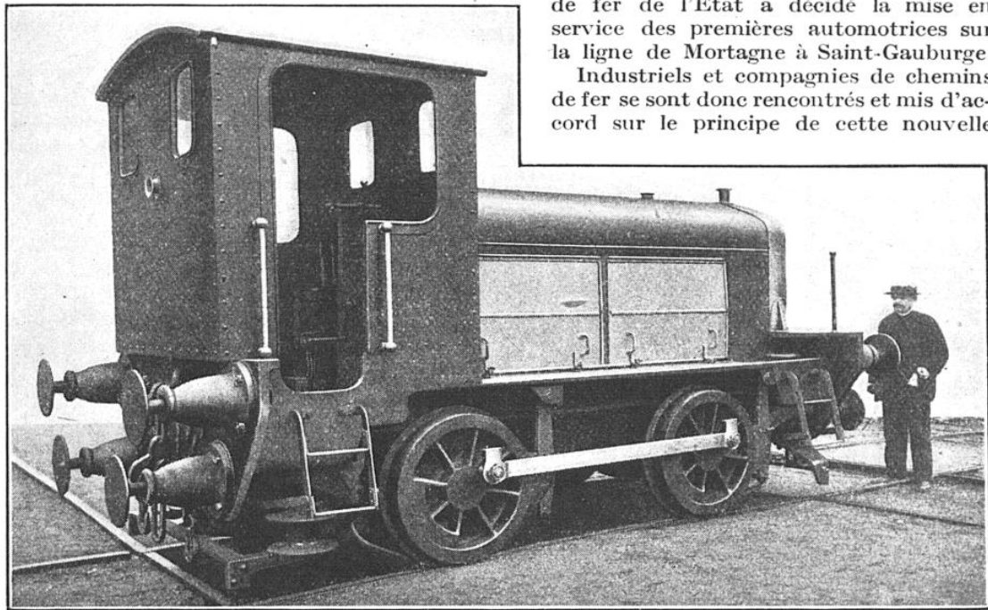
FIG. 12. — LOCOMOTIVE AÉROTHERMIQUE SYSTÈME HAUTIER ÉQUIPÉE AVEC UN MOTEUR A ESSENCE DE PÉTROLE DE 60 CHEVAUX
