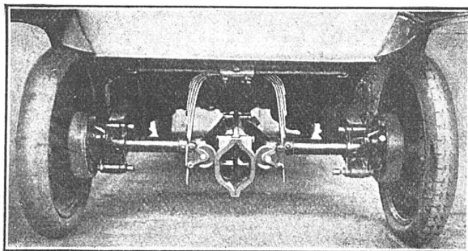
CONTRE-ACCÉLÉRATEUR « STAB » A L'ARRIÈRE D'UNE AUTO
