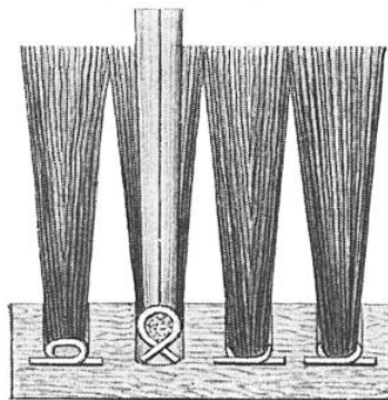
SYSTÈME DANS LEQUEL L'ANCRE EST REMPLACÉE PAR UNE AGRAFE EN FIL DE FER
