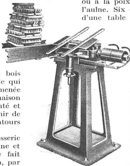
MACHINE A TONDRE METZLER, A COUTEAUX ROTATIFS, POUR ÉGALISER LA SURFACE DES SOIES
