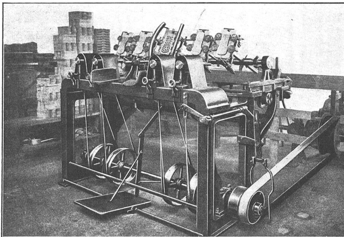
MACHINE A PERCER A QUATRE FORETS TRAVAILLANT EN MÊME TEMPS SUR QUATRE BOIS, CE QUI PERMET UNE FABRICATION TRÈS RAPIDE
