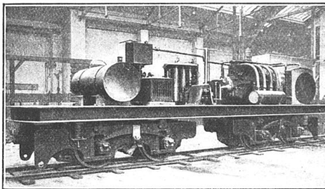
FIG. 10. — CHASSIS ÉQUIPÉ DE LA LOCOMOTIVE HENRY CROCHAT, DE 14 TONNES, EN SERVICE SUR UN GRAND NOMBRE DE VOIES FERRÉES MILITAIRES
