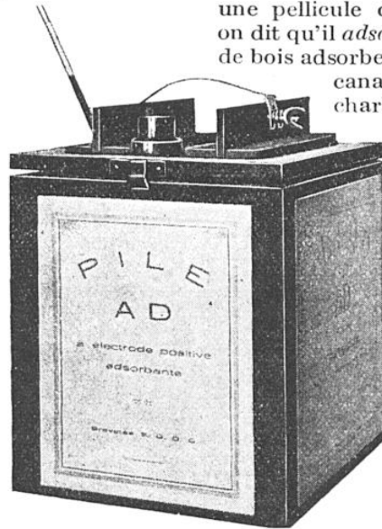
VUE EXTÉRIEURE DE LA PILE A DÉPOLARISATION AUTOMATIQUE
