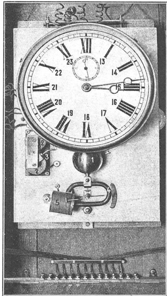
FIG. 3. — LE RÉGULATEUR
