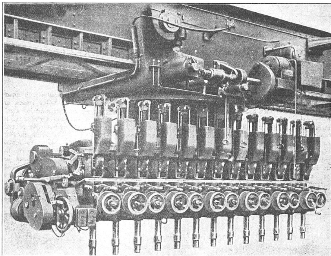
DÉTAIL DE LA TÊTE DE LA PERCEUSE GÉANTE A TREIZE FORETS
