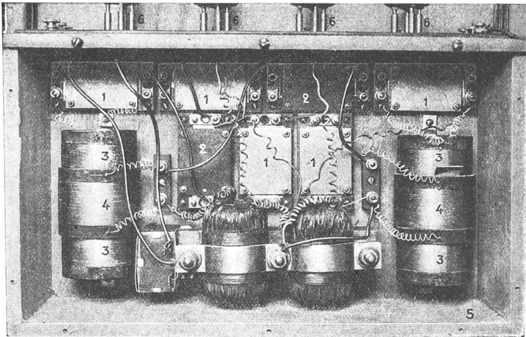
FIG. 7. — VUE GÉNÉRALE DES TRANSFORMATEURS
