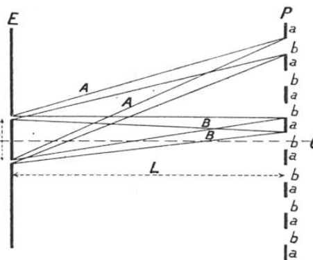
FIG. 7. - MESURE D'UNE LONGUEUR D'ONDE PAR LA DIFFRACTION
