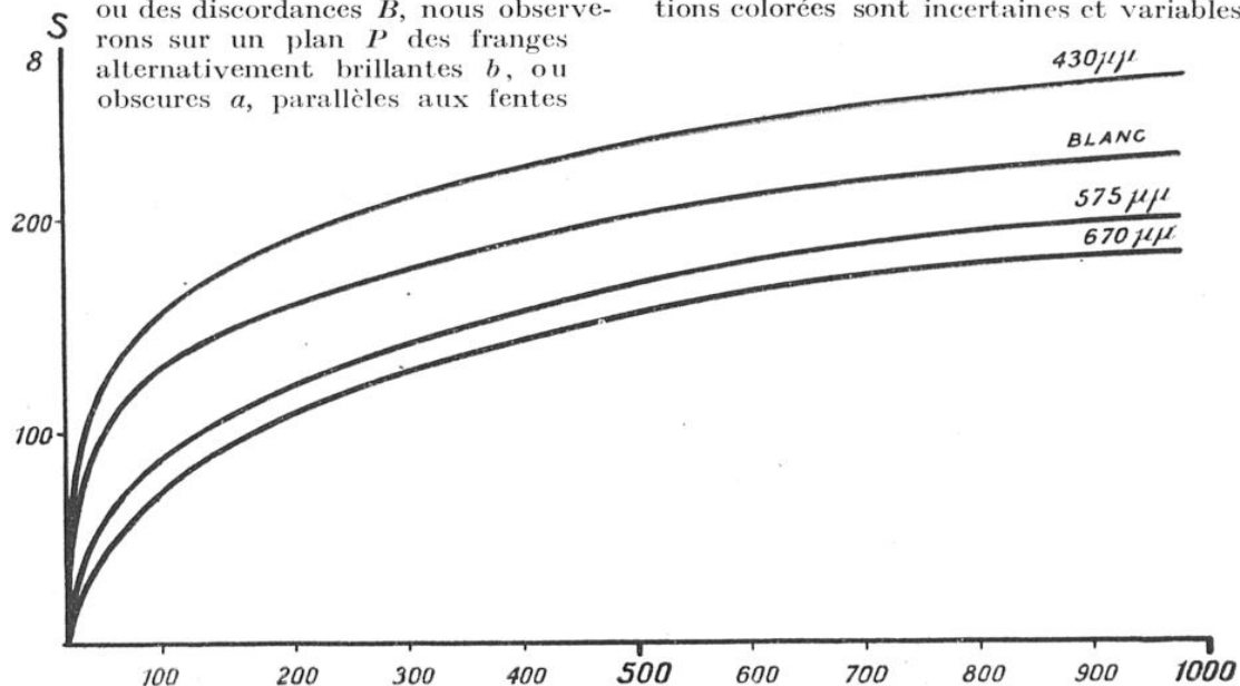
FIG. 8. — COURBES DES SENSATIONS EN FONCTION DES INTENSITÉS LUMINEUSES COLORÉES
