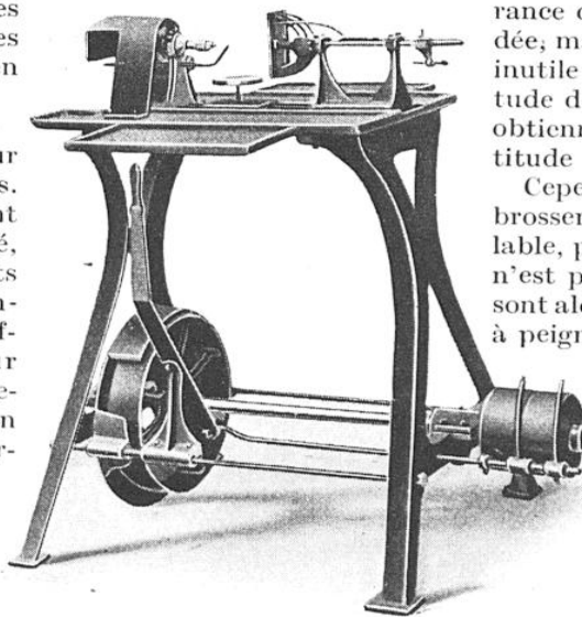
TOUR SIMPLE POUR PERCER LES BOIS
