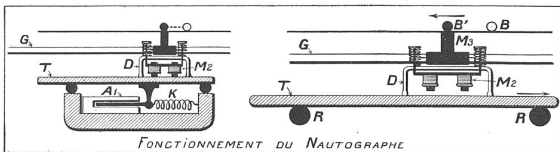
FIG. 6. — DÉTAILS DU FONCTIONNEMENT DU NAUTOGRAPHE
