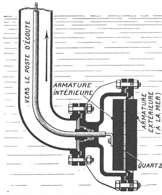
FIG. 1. — DIAPHRAGME PIEZO-ÉLECTRIQUE VU EN COUPE
