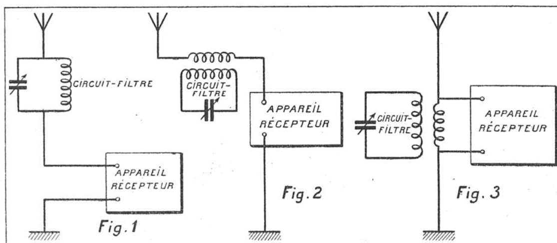
TROIS TYPES DE FILTRES QU'IL EST POSSIBLE DE RÉALISER FACILEMENT SOI-MÊME
