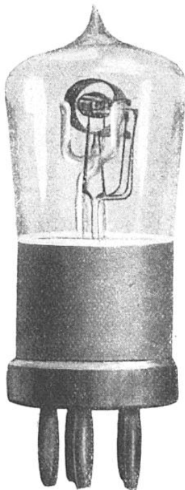
FIG. 12. — LAMPE ALLEMANDE A DEUX GRILLES
