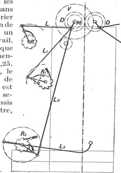
FIG. 2. — MÉCANISME DU NOUVEAU PILON
