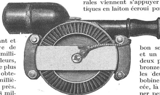
FIG. 2. — LA LAMPE « DE BOUCHE » DONT ON A ENLEVÉ LA TOLE PROTECTRICE POUR MONTRER LA TURBINE
