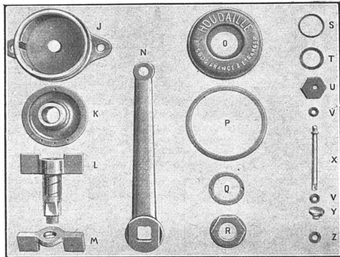
PIÈCES DÉTACHÉES CONSTITUANT LE CORPS DE L'AMORTISSEUR PROPREMENT DIT
