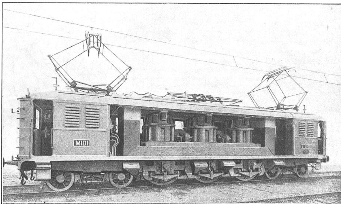
LOCOMOTIVE ÉLECTRIQUE A GRANDE VITESSE, TYPE 2. C. 2, DU MIDI Les panneaux latéraux ont été enlevés, et on aperçoit, à l'intérieur, les groupes de moteurs verticaux.
