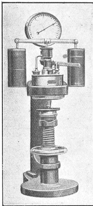
MACHINE A BILLES POUR L'ESSAI DES MÉTAUX
