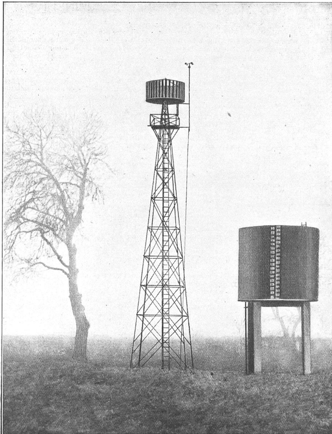
FIG. 1. — L'appareil est monté sur un terrain dégagé et il est équipé avec tous les instruments enregistreurs nécessaires (anémomètre, tachymètre, compteur de débit de pompe).
