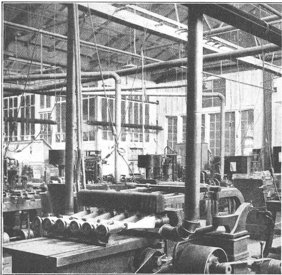
INSTALLATION DE CAPTATION DES SCIURES ET COPEAUX SUR DES MACHINES A FABRIQUER LES CROSSES DE FUSIL, DANS UNE MANUFACTURE DE L'ÉTAT
