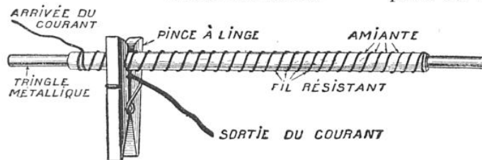
LA PINCE, DONT LE RESSORT MÉTALLIQUE EST RELIÉ AU CIRCUIT DANS LEQUEL ON VEUT FAIRE VARIER L'INTENSITÉ DU COURANT, SE COMPORTE COMME UN VÉRITABLE CURSEUR
