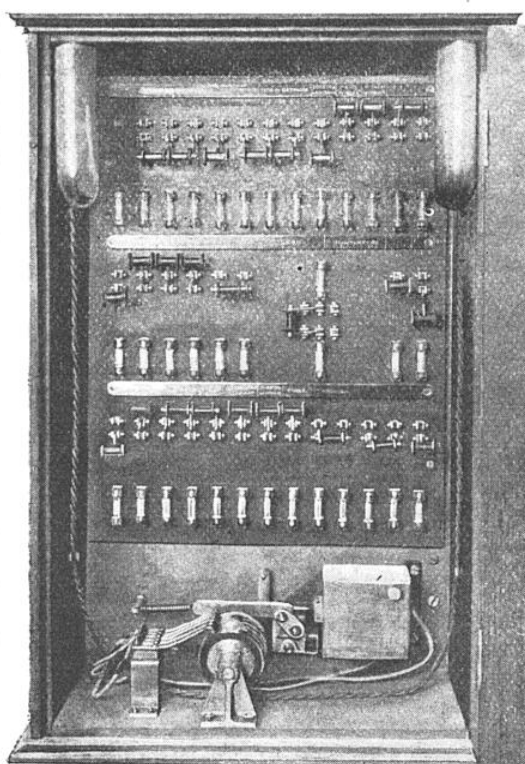
FIG. 9. — TABLEAU DE MANŒUVRE DE L'APPAREIL TRACEUR DE ROUTE
