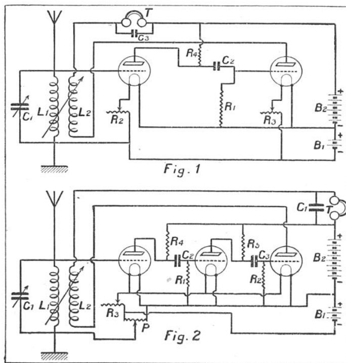
SCHEMAS DE MONTAGES A DEUX OU TROIS LAMPES AVEC COUPLAGE PAR RESISTANCES ET PAR CAPACITES
