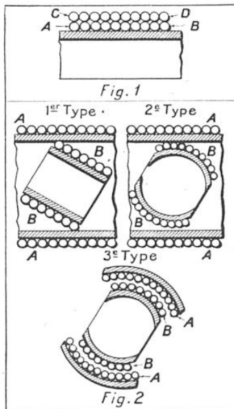
FIG. 1 : BOBINE A DEUX COUCHES ; FIG. 2 : TROIS TYPES COURANTS DE VARIOMÈTRES
