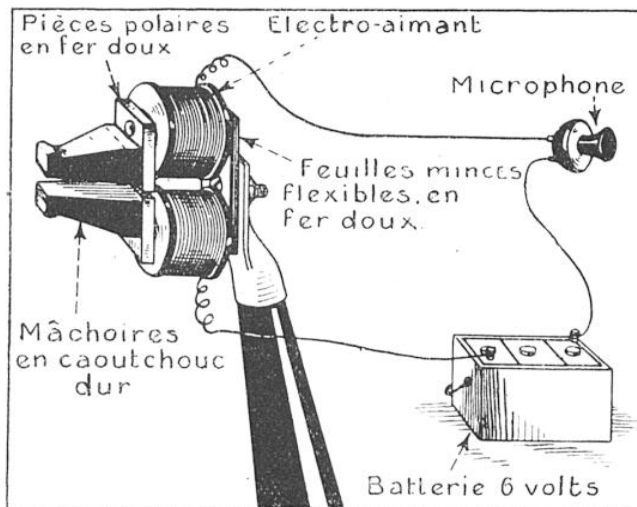
A gauche, détail de l'appareil ; à droite, l'inventeur utilisant l'Osophone pour « écouter » un concert radiotéléphonique.
