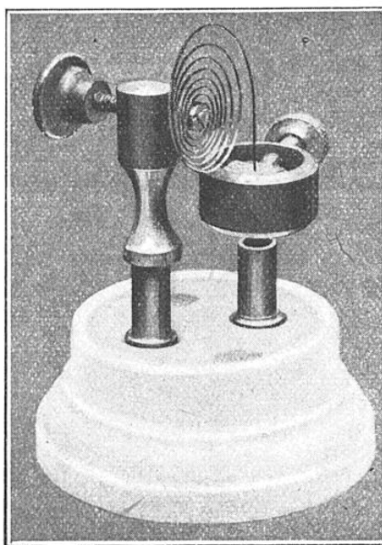
LE DÉTECTEUR « ROLLEX »
