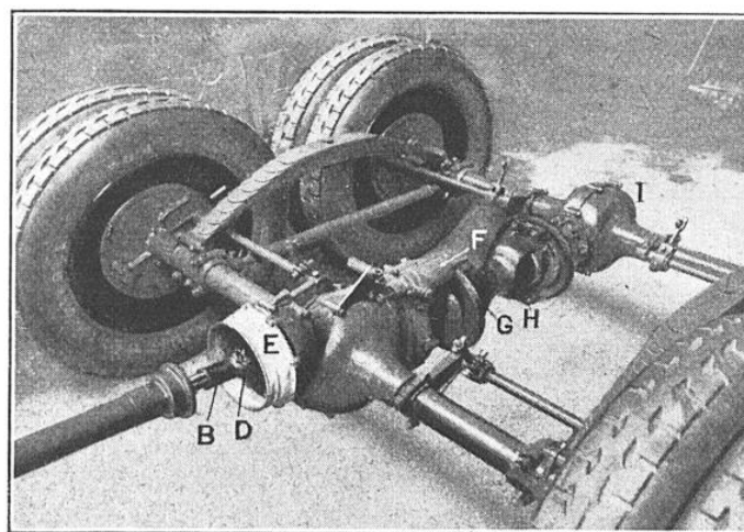
LA BOGIE-MOTEUR DE LA VOITURE
