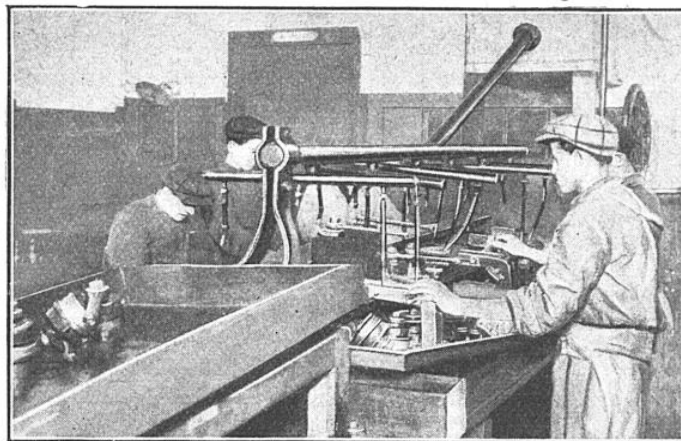
LE REMPLISSAGE D'HUILE DES BOITES D'AMORTISSEURS
