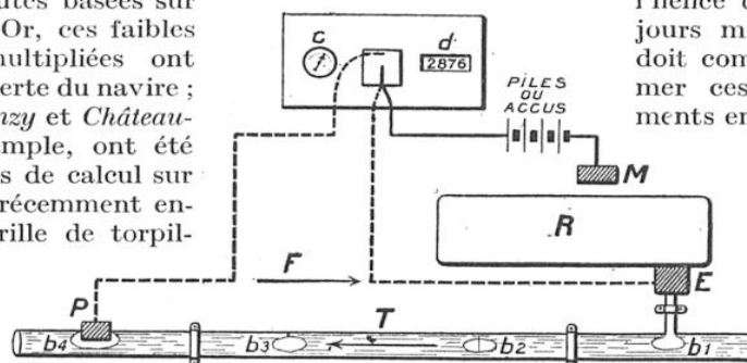
FIG. 2. — PRINCIPE DU LOCH ÉLECTRIQUE
