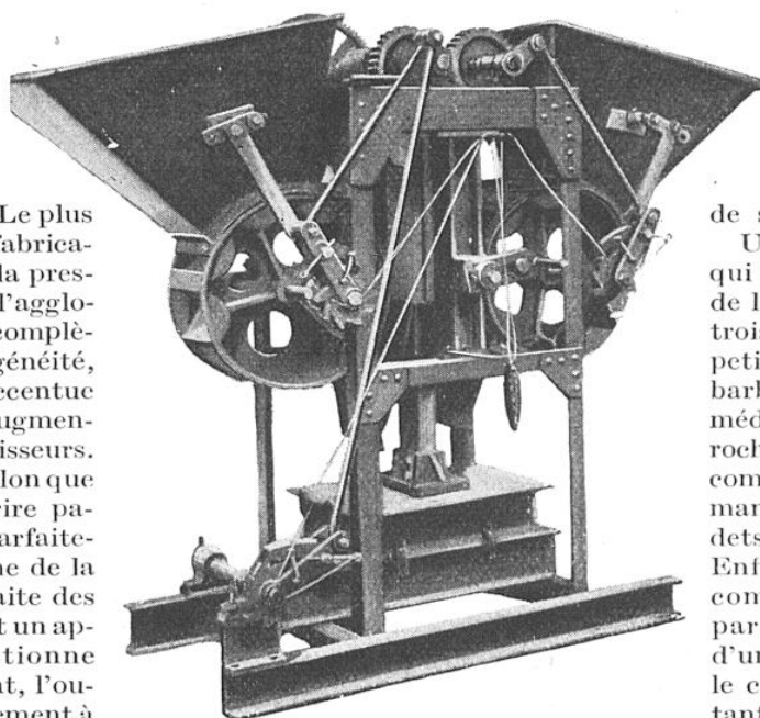
FIG. 1. — VUE GÉNÉRALE DU NOUVEAU PILON A AGGLOMÉRÉS
