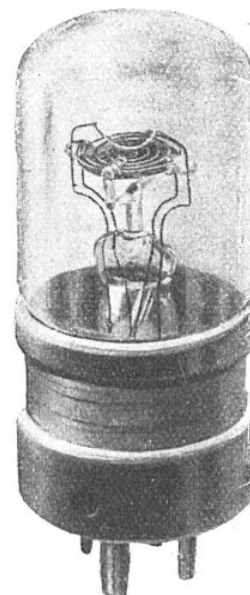
FIG. 10. — LAMPE ALLEMANDE, TYPE VERTICAL (TELEFUNKEN)
