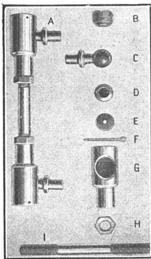
PIÈCES DÉTACHÉES DE LA TIGE DE LIAISON
