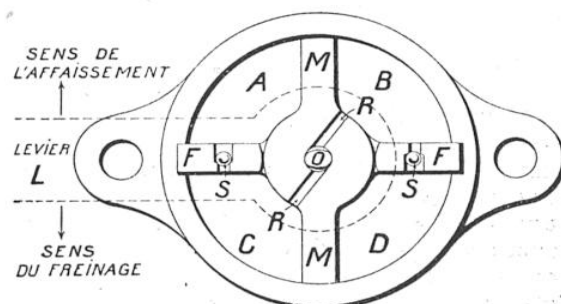
COUPE INTÉRIEURE DE L'AMORTISSEUR
