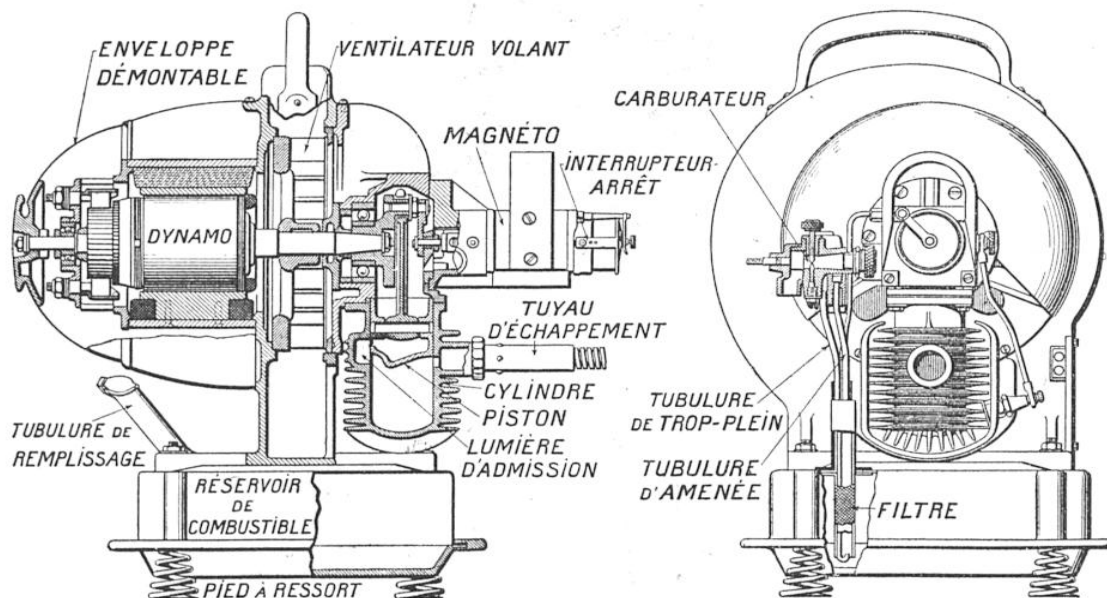
COUPE, PAR LE TRAVERS ET DE FACE, DU PETIT GROUPE ÉLECTROGÈNE « L'HOMELITE »
