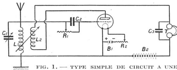
FIG. 1. — TYPE SIMPLE DE CIRCUIT A UNE SEULE LAMPE POUR ONDES LONGUES
