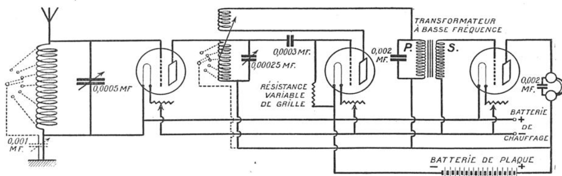
DISPOSITIF DU MONTAGE SIMPLE A RÉACTION ET A ANODE ACCORDÉE
