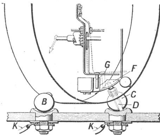
DÉTAIL DES CONNEXIONS ET CONTACTS ÉLECTRIQUES DU RÉVEIL PLACÉ SUR LE PLATEAU
