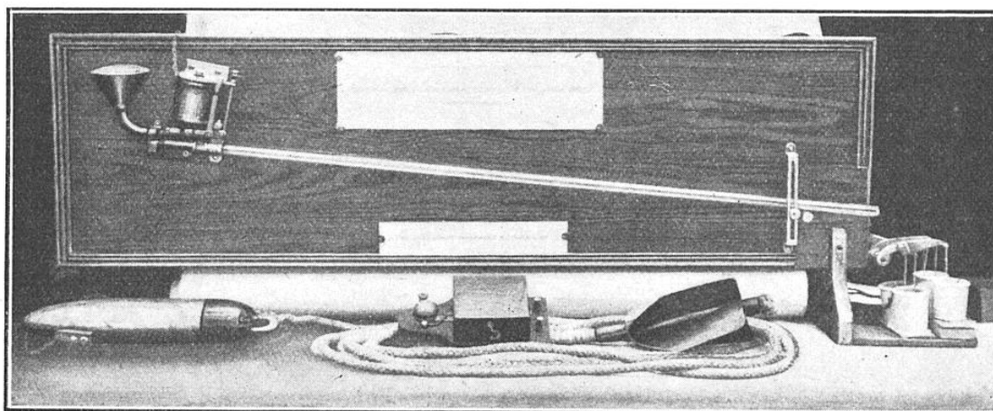
FIG. 4. — REPRÉSENTATION DU FONCTIONNEMENT DU LOCH BAULE A L'EXPOSITION DE PHYSIQUE DU GRAND PALAIS (DÉCEMBRE 1923)
