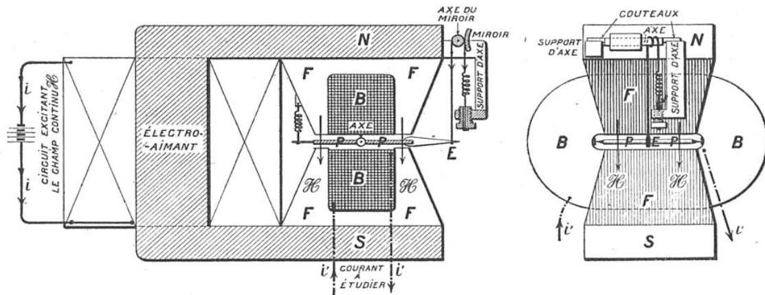
FIG. 6. — COUPE DE L'OSCILLOGRAPHÉ ÉLECTROMAGNÉTIQUE DE M. R. DUBOIS
