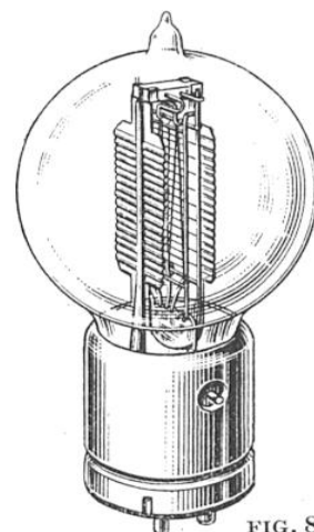
FIG. 8 LAMPE A FILAMENT OUTRE, RECOUVERT D'OXYDES SUR LA (WESTERN-ELECTRIC) figure, la forme spéciale de la plaque, formée d'anneaux superposés.
