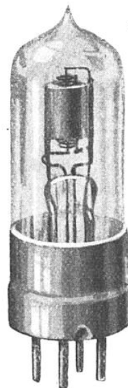
FIG. 3. — LAMPE ANGLAISE A ÉLECTRODES VERTICALES
