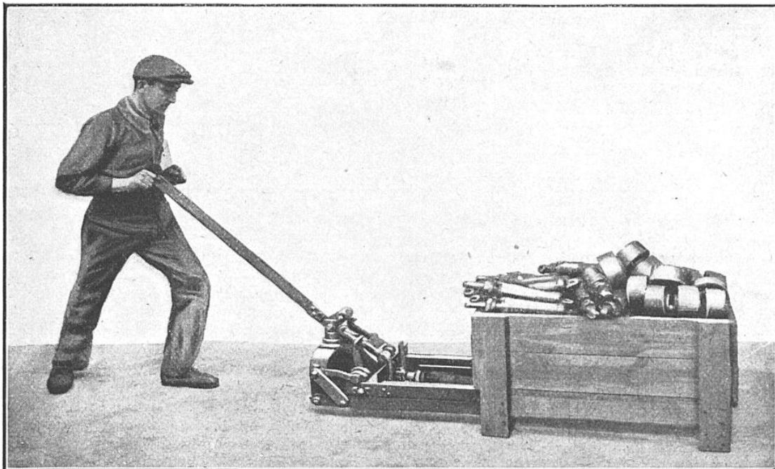
COMMENT ON UTILISE LE NOUVEAU CHARIOT ÉLEVATEUR
