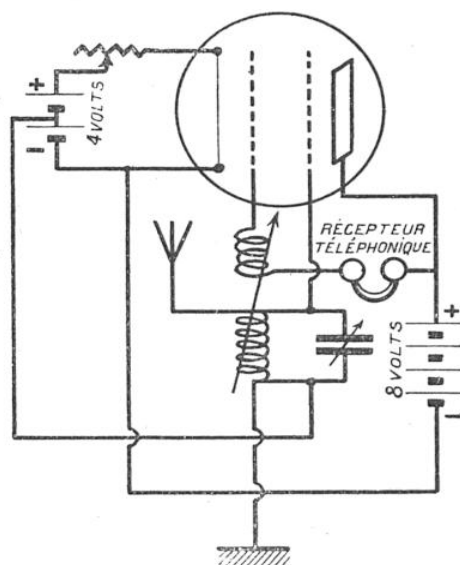
FIG. 15. — MONTAGE D'UNE LAMPE A DEUX GRILLES A DÉTECTRICE AUTODYNE
