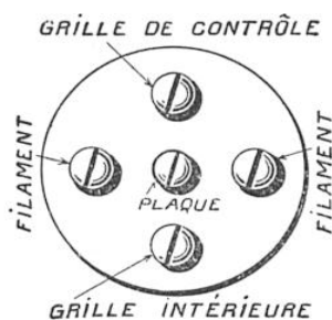
FIG. 14. — COMMENT SE PRÉSENTE LE CULOT D'UNE LAMPE A DEUX GRILLES
