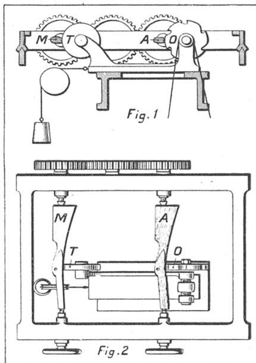
SCHEMAS DE LA MACHINE A FABRIQUER LES CROSSES DE FUSIL
