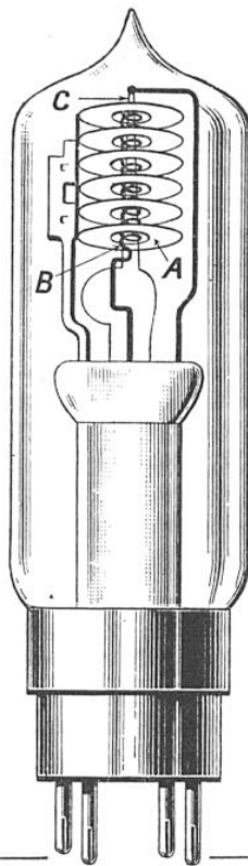
FIG. 11. — LE TRIODE « JUNOT » A DEUX FILAMENTS
