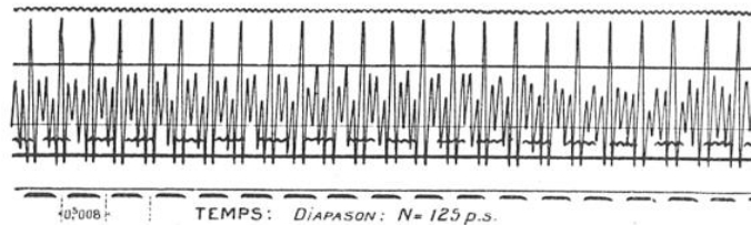
FIG. 8. — OSCILLOGRAMME D'UN COURANT TÉLÉPHONIQUE (VOYELLE O)
