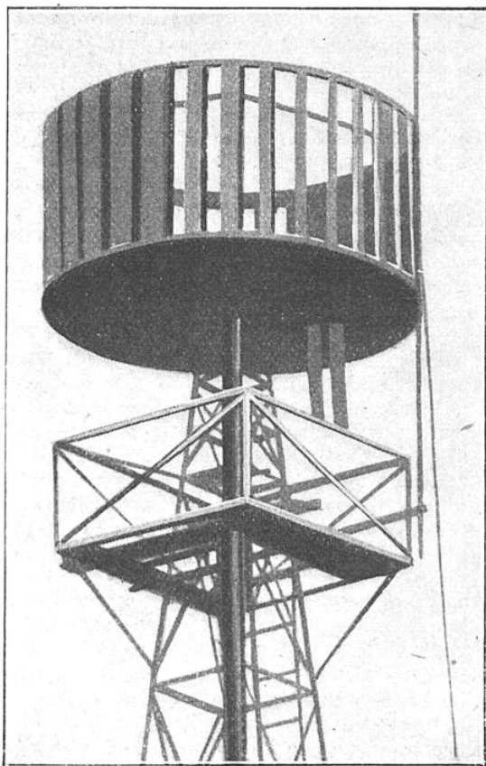
FIG. 5. — TAMBOUR ROTATIF DE LA TURBINE AÉRIENNE (MODÈLE PRIMITIF)
