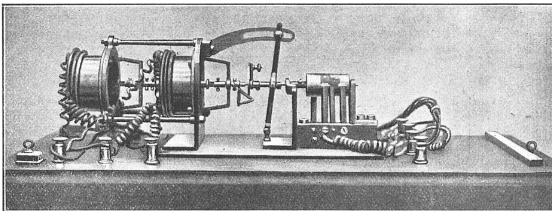
FIG. 7. — DISTRIBUTEUR DE CAP, SOLIDAIRE DU TRACEUR DE ROUTE C'est l'appareil de remplacement du compas gyroscopique.
