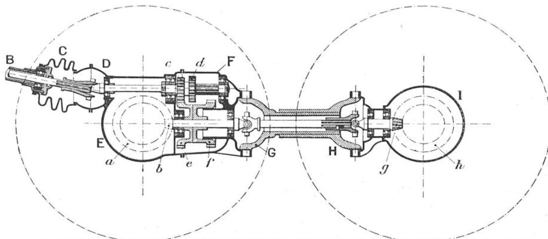
COUPE SCHÉMATIQUE DE LA TRANSMISSION AUX DEUX PONTS-MOTEUR
