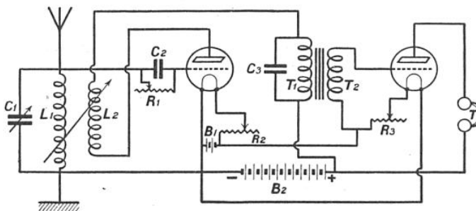
FIG. 2. — MONTAGE DU CIRCUIT AUGMENTÉ D'UNE SECONDE LAMPE
