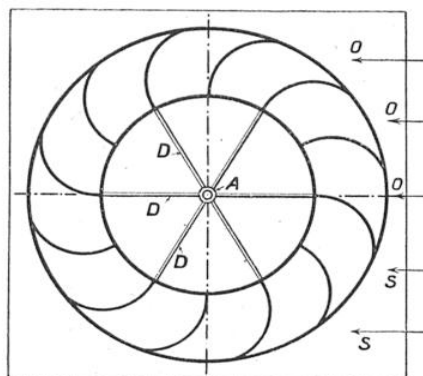
FIG. 6. — SCHÉMA DE FONCTIONNEMENT DU TAMBOUR ROTATIF
