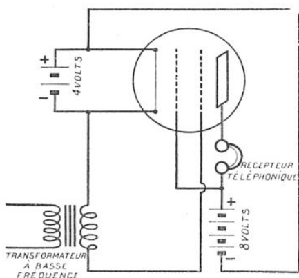
FIG. 16. — LAMPE A DEUX GRILLES MONTÉE EN AMPLIFICATRICE A BASSE FRÉQUENCE
