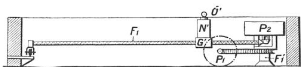
FIG. 10. — RÉPÉTITEUR DES INDICATIONS FOURNIES PAR LE NAUTOGRAPHE
