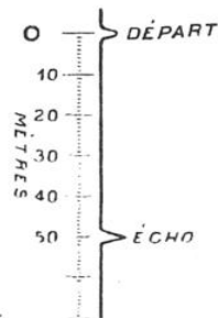
FIG. 9. — SCHÉMA DE LA RÉCEPTION OPTIQUE DES ULTRA-SONS
