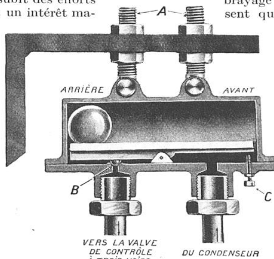
FIG. 1. — COUPE LONGITUDINALE DE LA BOITE CONTENANT LA BILLE ET LA VALVE RAMSAY
