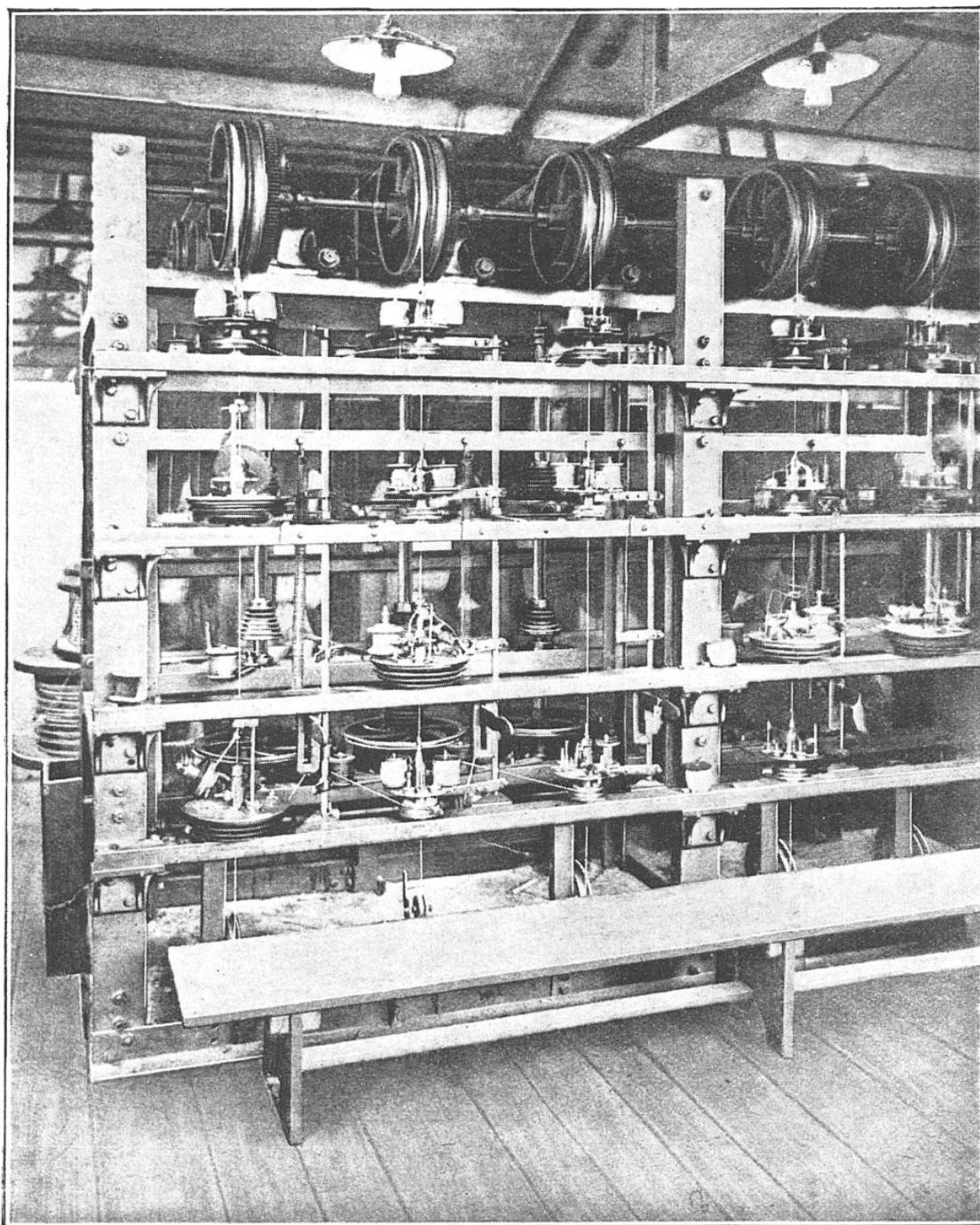
FIG. 2. — MACHINE A GUIPER, C'EST-A-DIRE A RECOUVRIR DE COTON, DE PAPIER OU DE RUBAN LES FILS DE CUIVRE APPARTENANT AU TYPE DIT DE SONNERIE
