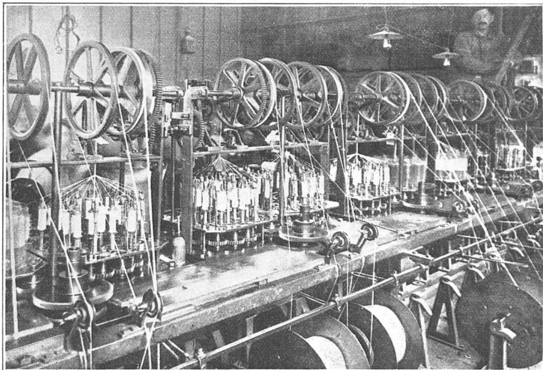
FIG. 15. — TRESSEUSE A VINGT-QUATRE FUSEAUX (LE FONCTIONNEMENT DE CETTE MACHINE EST EXPLIQUÉ PAR LES DESSINS SCHÉMATIQUES 16 ET 17)
