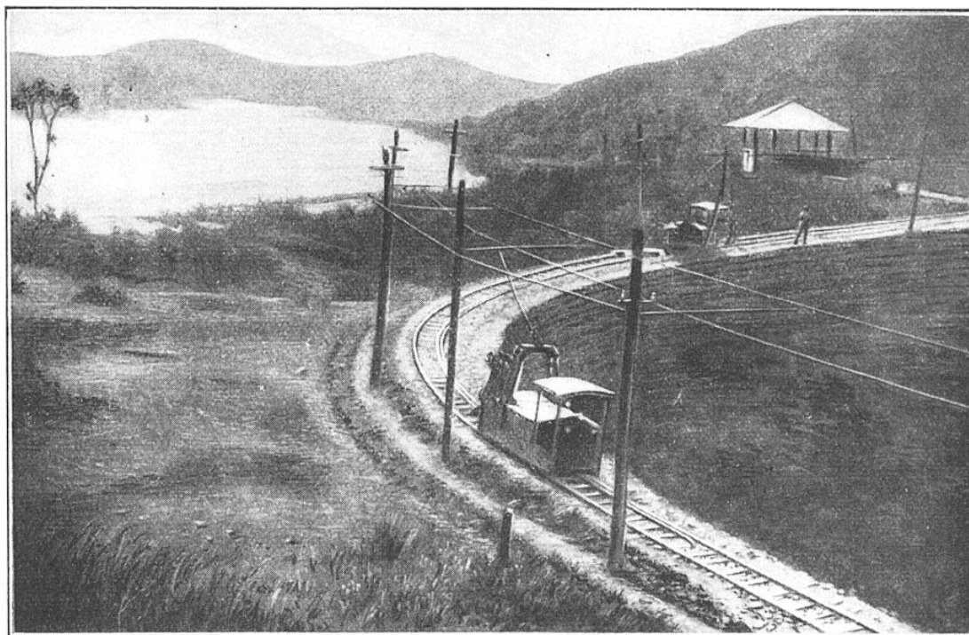
SECTION DU CHEMIN DE FER ÉLECTRIQUE DE JITSUGETSUTAN (ILE DE FORMOSE)
