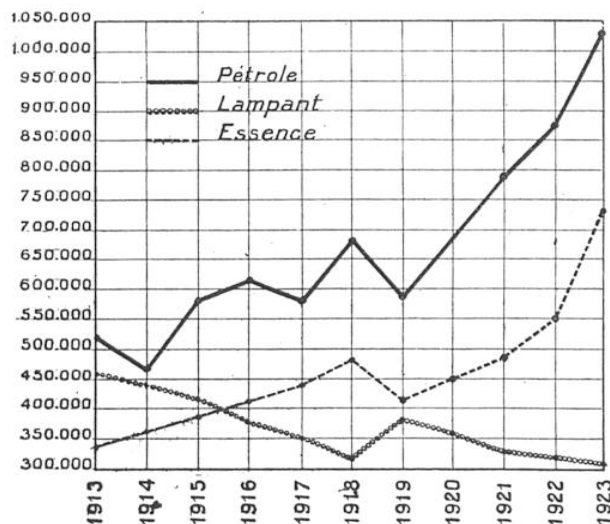
IMPORTATION DU PÉTROLE EN FRANCE ET IMPORTATION COMPARÉE DU PÉTROLE ET DE L'ESSENCE (EN TONNES)
