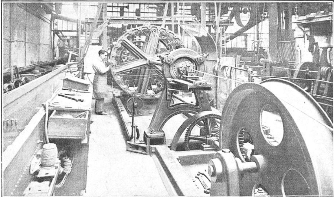
FIG. 14. — MACHINE A DÉTORSION DE VINGT-QUATRE BOBINES UTILISÉE POUR LA FABRICATION DES GROS CABLES (CETTE MACHINE EST SCHÉMATISÉE DANS LA FIGURE 13)
