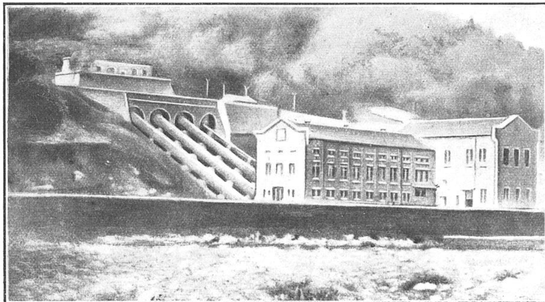
USINE D'OKUWA, SUR LA RIVIÈRE KISO, EN AVAL DE SUHARA
