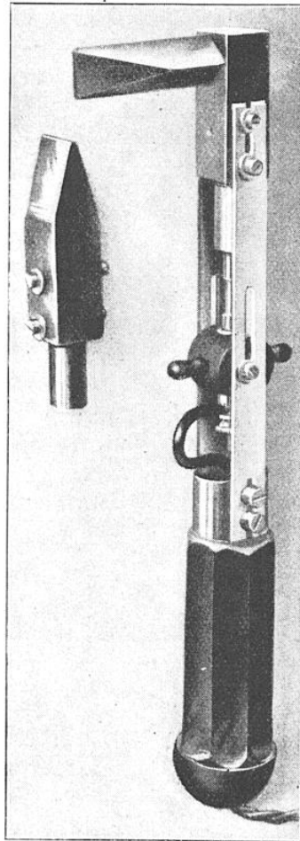
LE FER A SOUDER « ARCTURUS » En haut et à gauche, la tête droite qui peut remplacer celle en équerre.
