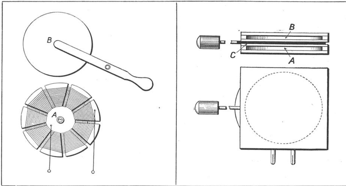
FIG. 7. — MÉTHODE SIMPLE POUR FAIRE VARIER L'INDUCTANCE DE LA BOBINE « A » AU MOYEN D'UNE PLAQUE MÉTALLIQUE « B » MOBILE PAR RAPPORT A LA BOBINE
