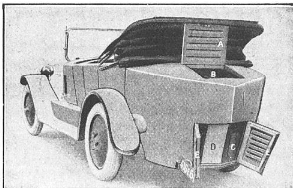
LE GAZOGÈNE IMBERT DISPOSÉ À L'ARRIÈRE D'UNE VOITURE BERLIET
