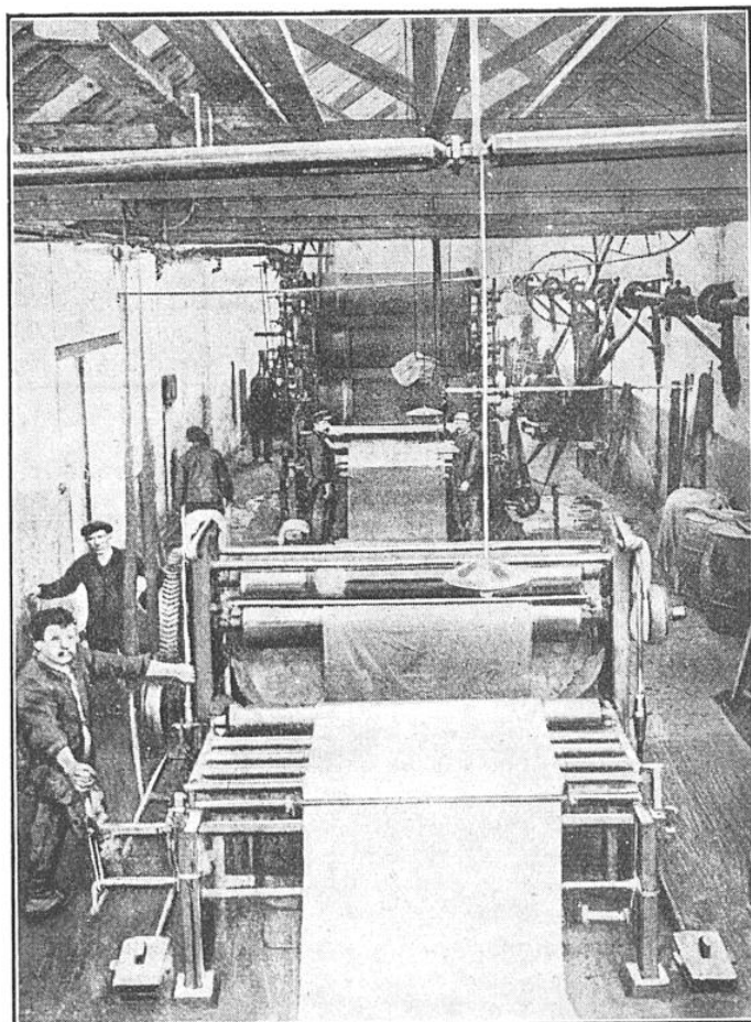
VUE DE FACE D'UN « MÉTIER » A IMPERMÉABILISER AU MOYEN DE L'ACÉTATE D'ALUMINE OU DE TOUTE AUTRE COMPOSITION CHIMIQUE ÉQUIVALENTE
