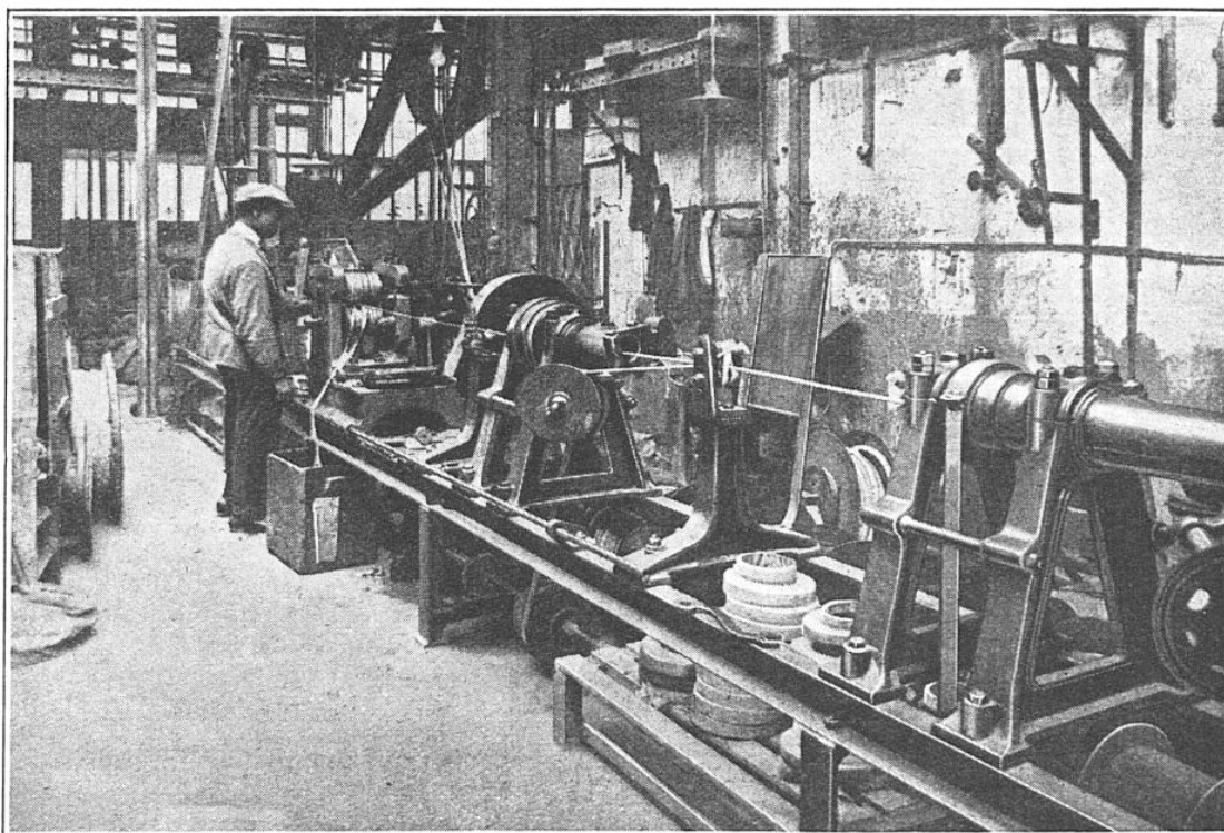
FIG. 3. — MACHINE A GALETS POUR GROS CABLES, ISOLANT UN SEUL CABLE PAR LA SOUDURE DES BANDES DE CAOUTCHOUC
