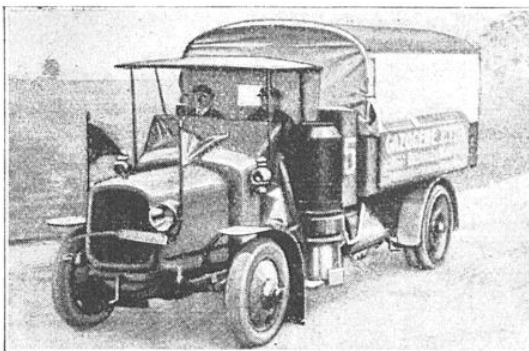
Le Gazogène ÉTIA alimentant un camion 4 tonnes Delahaye au Concours de l'A. C. F.
