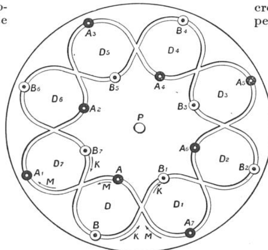
FIG. 16 ET 17. — MACHINE A TRESSER
