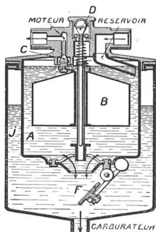
COUPE DE L'ÉLÉVATEUR D'ESSENCE
