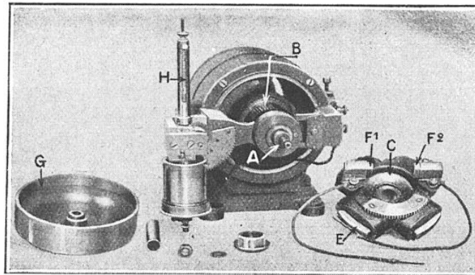
FIG. 2. — DÉTAILS DE LA DYNAMO A TENSION CONSTANTE
