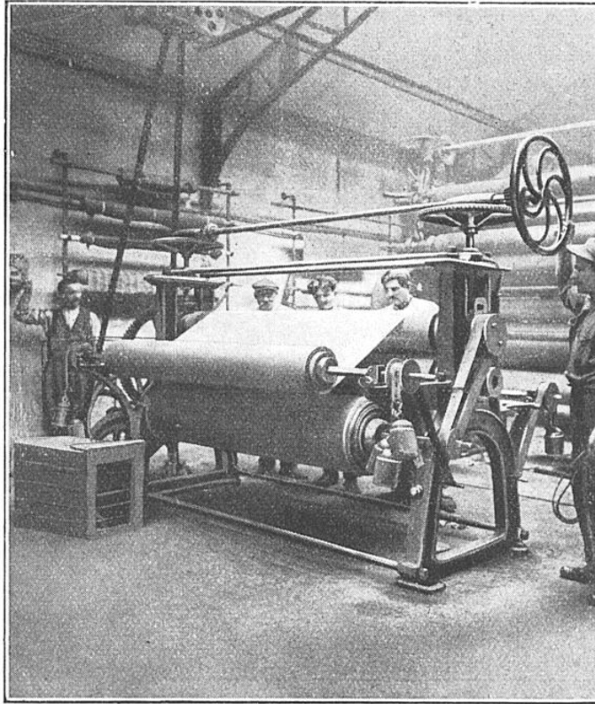
MACHINE A DOUBLER LES TISSUS, DITE « DOUBLEUSE » Pour doubler les tissus, on les passe, en mettant leur surface caoutchoutée en contact, entre deux cylindres qui les pressent assez fortement l'un contre l'autre pour opérer leur collage.
