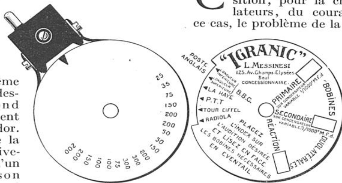
LE TABLEAU-DISQUE « IGRANIC » POUR DÉTERMINER IMMÉDIATEMENT LES INDUCTANCES
