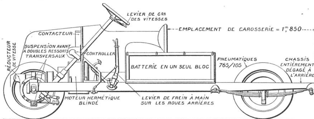
VUE EN COUPE DU CHASSIS DE LA SOCIÉTÉ D'APPLICATIONS ÉLECTROMÉCANIQUES, AVEC L'ESSIEU AVANT MOTEUR ET DIRECTEUR
