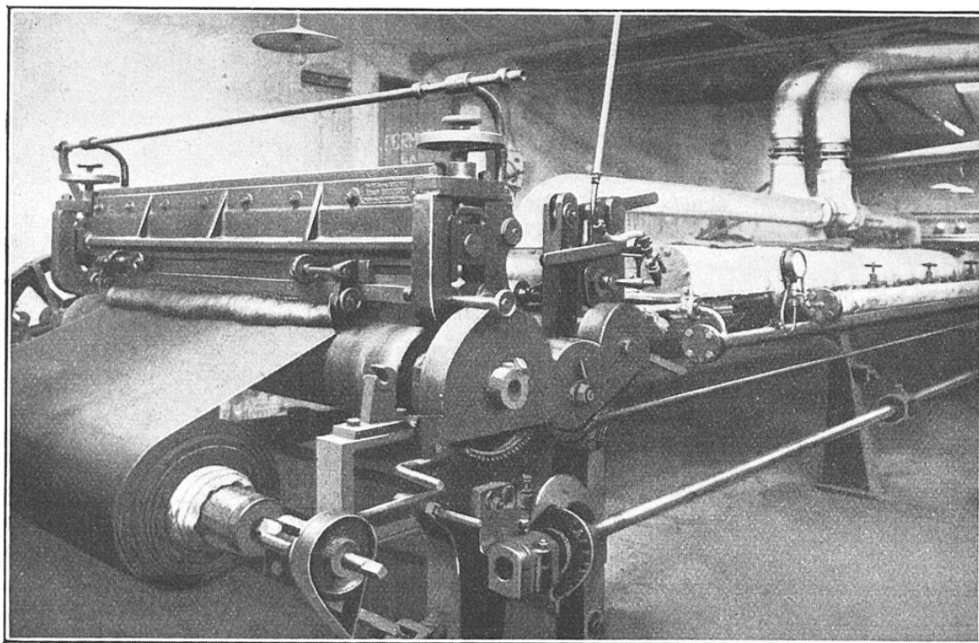
VUE DE L'UNE DES EXTRÉMITÉS D'UNE MACHINE A IMPERMÉABILISER, DITE « MÉTIER »
