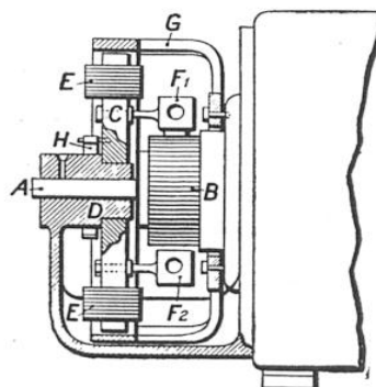
FIG. 4. — AUTRE DISPOSITIF DE LA CLOCHE ET DU PORTE-BALAIS MOBILES
