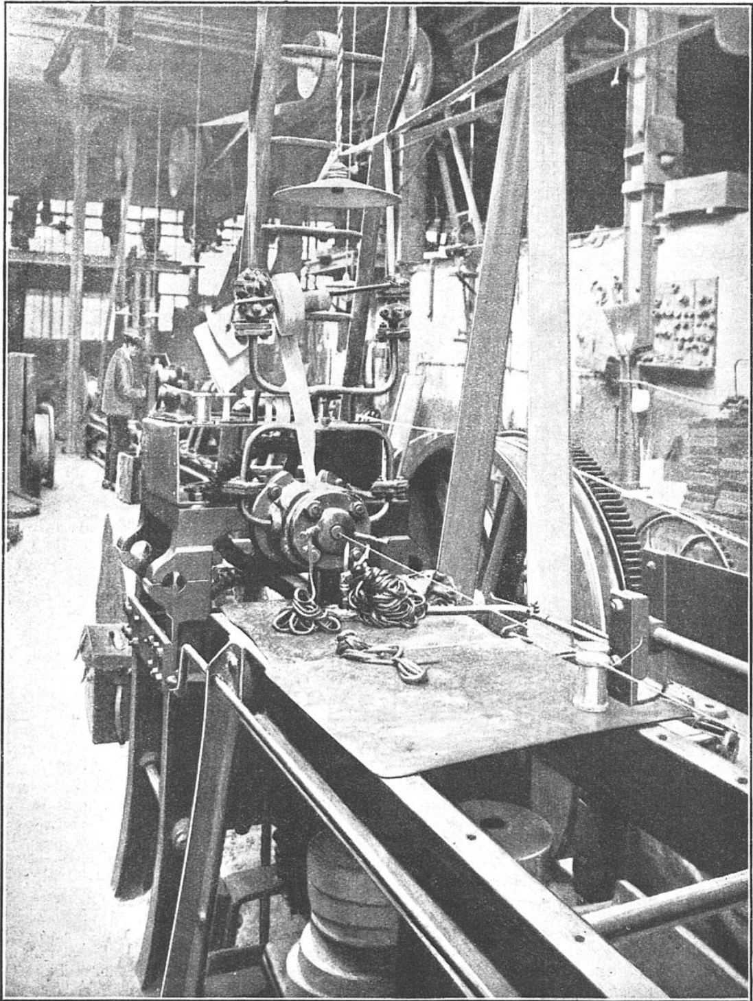
FIG. 6. — MACHINE A VIS HÉLICOIDALE SCHÉMATISÉE DANS LA FIGURE 7 Cette machine est destinée à recouvrir de caoutchouc, par pression, les fils et les câbles. La bobine sur laquelle est enroulé le caoutchouc est disposée au-dessus de la machine et laisse tomber le ruban dans le réservoir contenant l'isolant.
