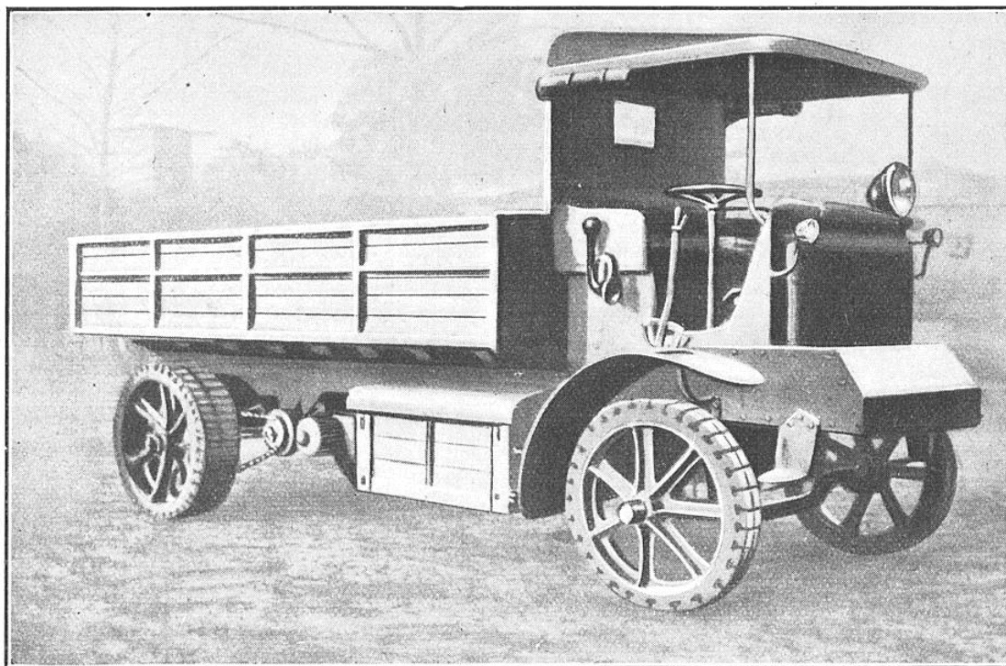
CAMION A ACCUMULATEURS ÉLECTRIQUES, SYSTÈME CROCHAT
