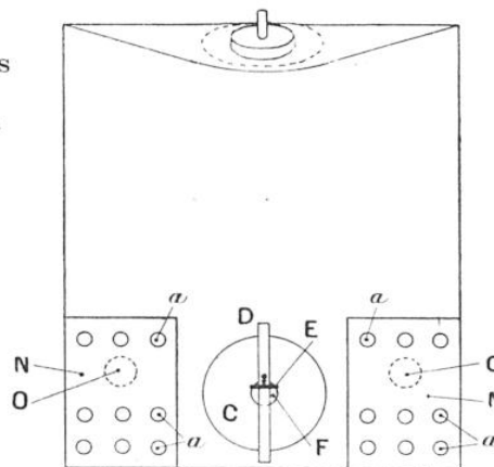
COUPES SCHÉMATIQUES DU GÉNÉRATEUR IMBERT
