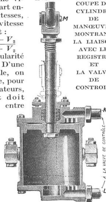
K, L, Orifices de communication avec la valve de contrôle; M, axe d'articulation avec la transmission au registre.
