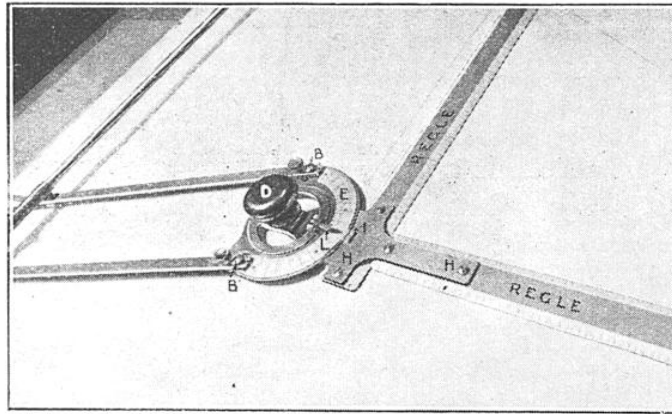
DÉTAIL DE LA NOUVELLE MACHINE A DESSINER
