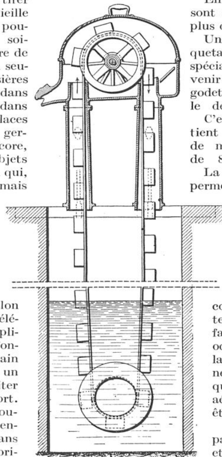
COUPE DE L'ÉLÉVATEUR « DRAGOR »
