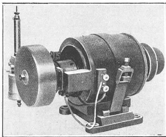
FIG. 1. — DYNAMO D'ÉCLAIRAGE A TENSION CONSTANTE
