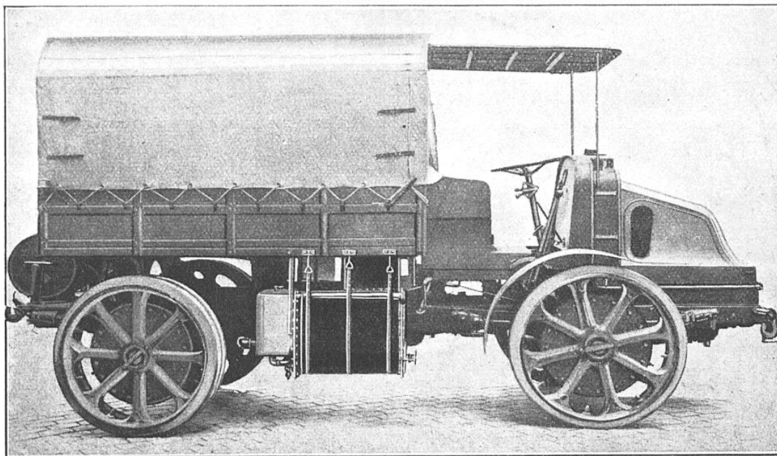
LE GAZOGÈNE MIS EN PLACE SUR UN CAMION AUTOMOBILE
