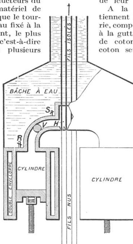
FIG. 1. — SCHÉMA DE LA MACHINE A DÉPOSER DE LA GUTTA-PERCHA SUR LES FILS
