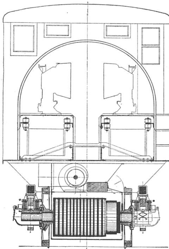
VUE DE L'INDUIT, ET, PARTIELLEMENT, DE L'INDUCTEUR D'UN ESSIEU MOTEUR
