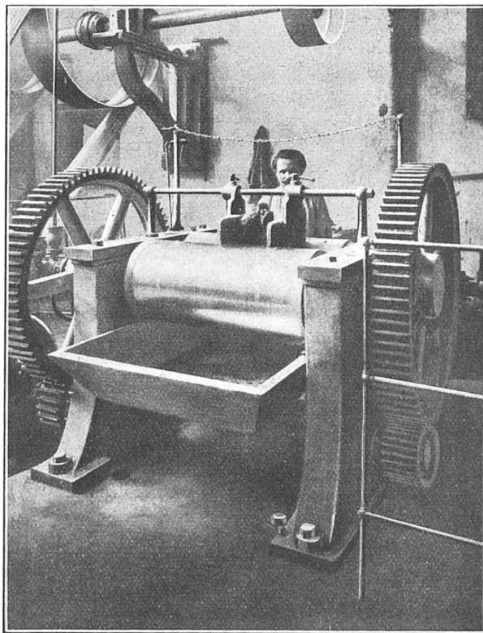
MÉLANGEUSE VUE DE FACE
