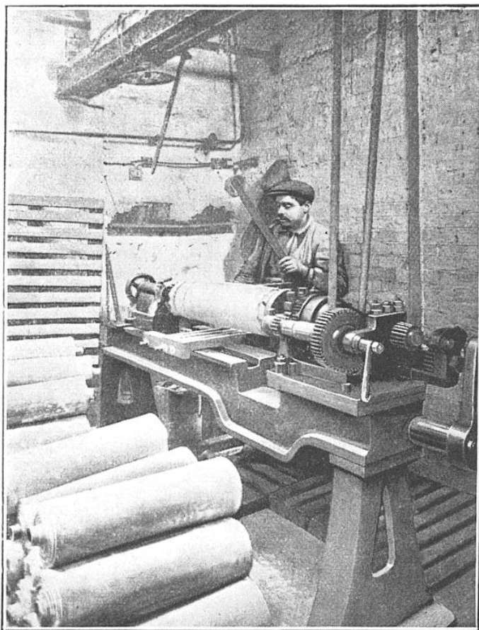
FIG. 8. — TOUR DESTINÉ A COUPER LE CAOUTCHOUC EN BANDES DE DIVERSES LARGEURS
