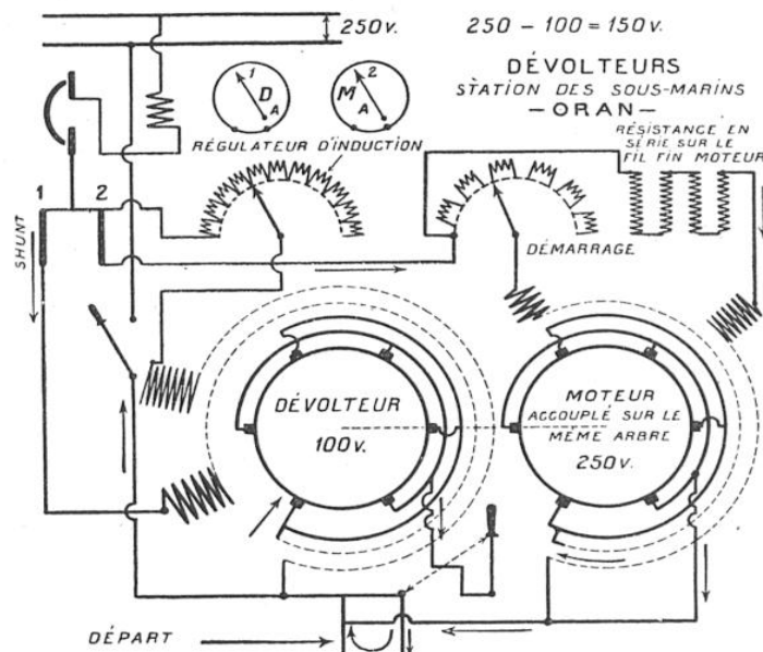
FIG. 2. — SCHÉMA EXPLICATIF D'UN GÉNÉRATEUR-DÉVOLTEUR
