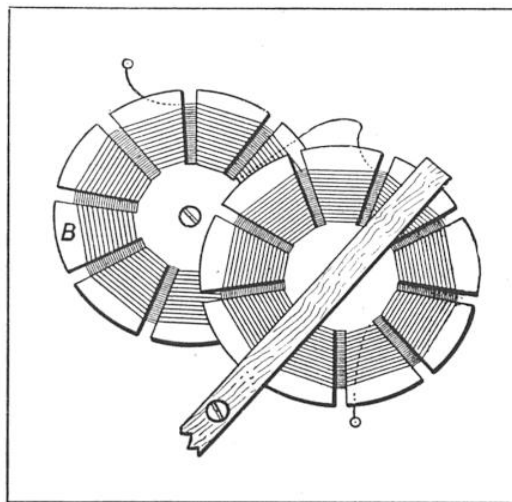
FIG. 9. — LA FORME LA PLUS SIMPLE DE VARIOMÈTRE CONSISTE EN DEUX BOBINES EN FOND DE PANIER CONNECTÉES EN SÉRIE, L'UNE ÉTANT MOBILE PAR RAPPORT A L'AUTRE « B »
