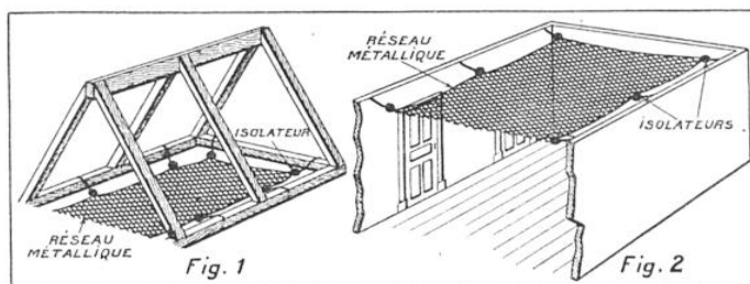
FIXATION DES RÉSEAUX MÉTALLIQUES EMPLOYÉS COMME ANTENNE
