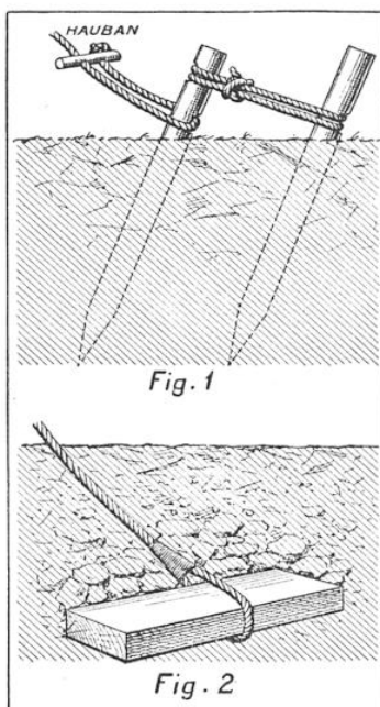
DEUX MODES D'ANCRAGE DES HAUBANS DE MÂTS
