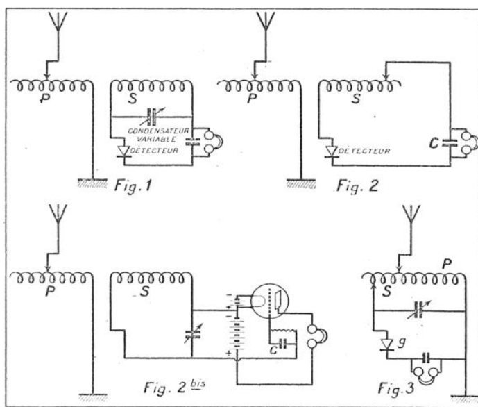
MONTAGES POUR LA RÉCEPTION DES ONDES COURTES PAR CIRCUITS À RÉSONANCE
