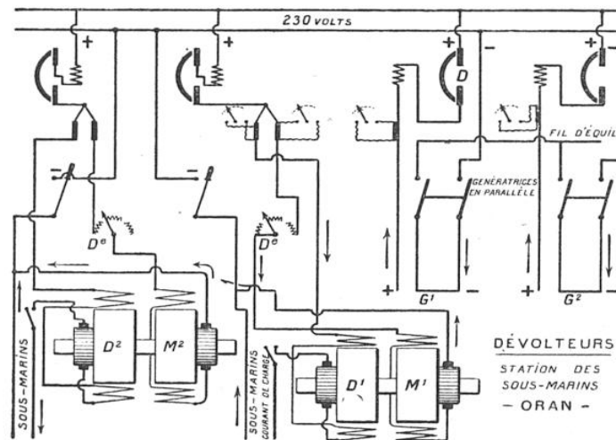
FIG. 1. — GÉNÉRATEURS-DÉVOLTEURS DE LA STATION DES SOUS-MARINS D'ORAN
