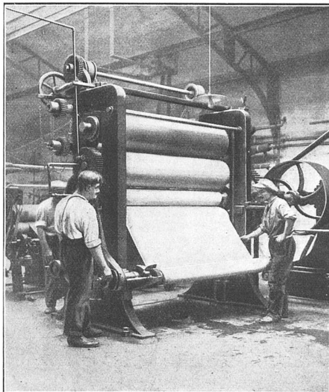
CALANDRE DANS LAQUELLE LE TISSU CAOUTCHOUTÉ EST PASSÉ POUR DONNER A SA SURFACE UN POLI PARFAIT
