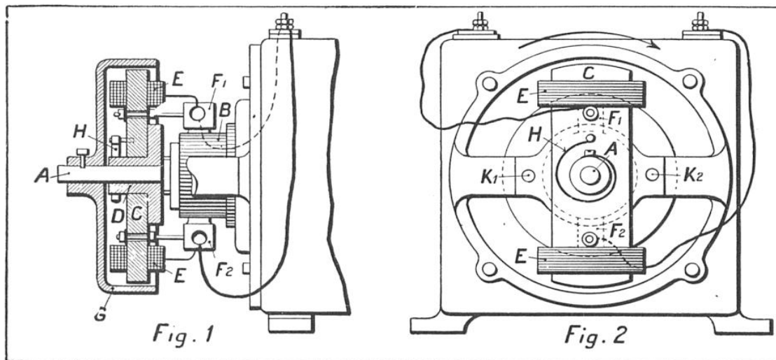
PLANCHE 3. — COUPES DE LA DYNAMO A POTENTIEL CONSTANT
