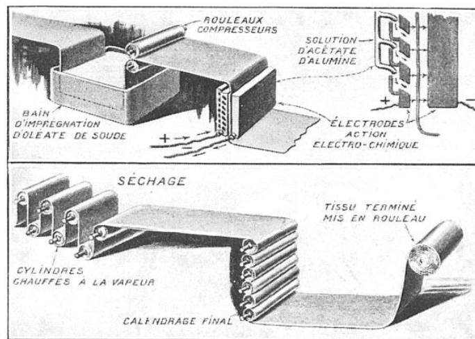
VUE SCHÉMATIQUE D'UN DISPOSITIF POUR L'IMPERMÉABILISATION DES TISSUS PAR LE PROCÉDÉ ÉLECTRO-CHIMIQUE
