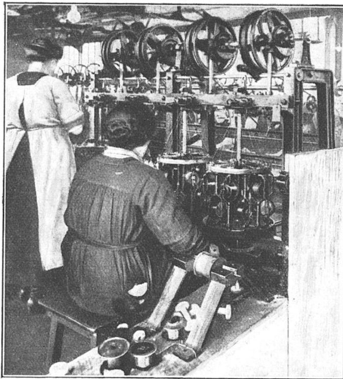
FIG. 12. — PETITE CÂBLEUSE A DÉTORSION POUR FABRIQUER DES CÂBLES TRÈS SOUPLES A FILS EXTRÊMEMENT FINS
