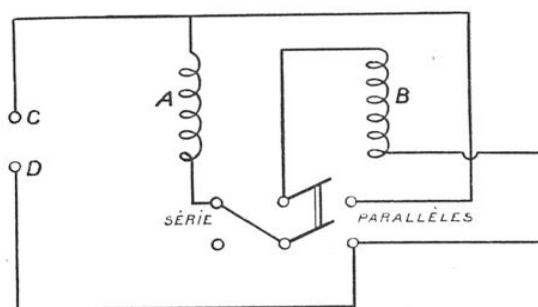
FIG. 6. — MÉTHODE DE CONNEXION EMPLOYANT UN COMMUTATEUR POUR LE FONCTIONNEMENT DES BOBINES EN SÉRIE OU EN PARALLÈLE
