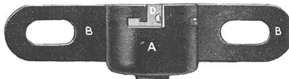
PIÈCES COMPOSANT LA LANTERNE
