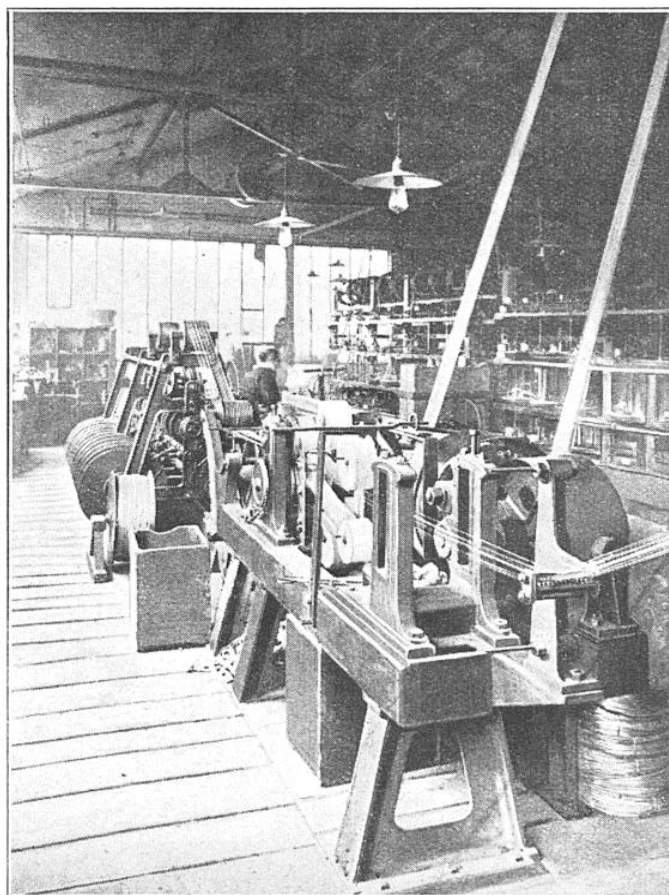
FIG. 5. — MACHINE A GALETS A DOUZE FILS ISOLANT, SOUS CAOUTCHOUC A FROID, PLUSIEURS FILS A LA FOIS EN SOUDANT LES BANDES DE CAOUTCHOUC (La figure 4 en représente également le principe.)
