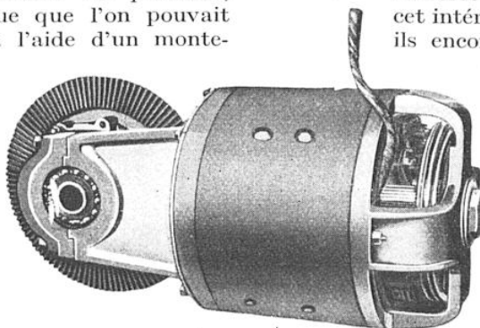
ENSEMBLE DU MOTEUR MONTÉ DIRECTEMENT SUR LE PONT-ARRIÈRE, DONT LA BOÎTE CONTENANT LE COUPLE CONIQUE ET LE DIFFÉRENTIEL EST À DÉCOUVERT
