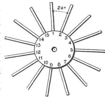
TYPE DE MANDRIN POUR BOBINES EN PANIER
