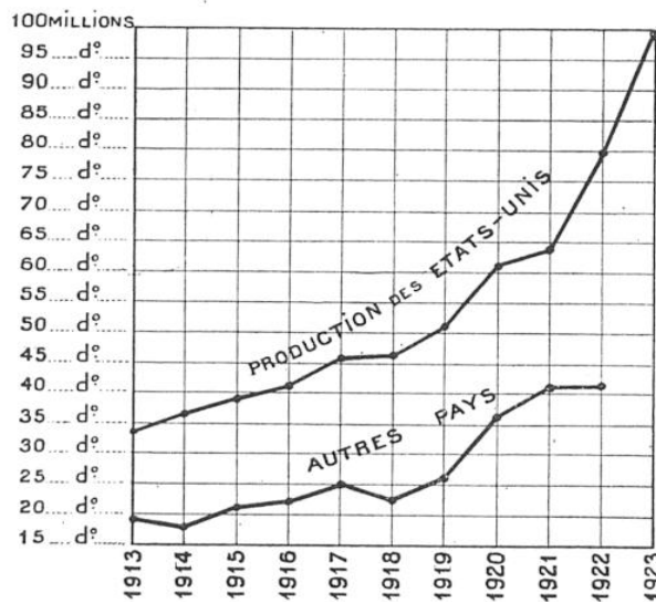
LA PRODUCTION DU PÉTROLE BRUT AUX ÉTATS-UNIS ET DANS LES AUTRES PAYS, EXPRIMÉE EN TONNES
