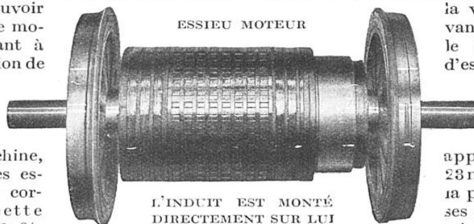
Chaque essieu moteur pèse, avec ses deux roues et l'induit, environ 4.220 kilos. La puissance totale des douze moteurs atteint, en régime normal, 2.760 chevaux-vapeur pour un effort de traction moyen de 19 tonnes.
