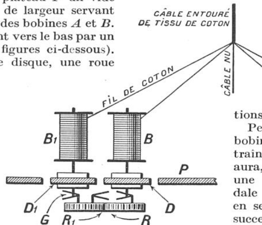
FIG. 16 ET 17. — MACHINE A TRESSER
