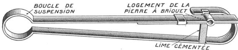
CE BRIQUET NE COMPORTE NI VIS, NI RIVET, NI ARTICULATION
