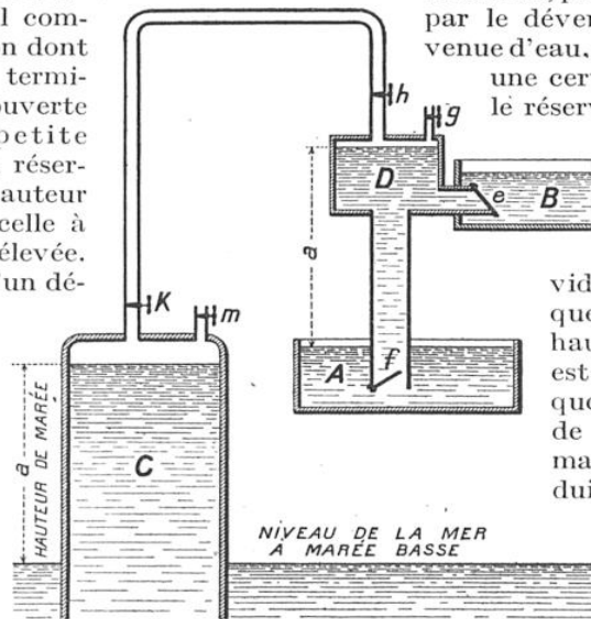
LE SYSTÈME DE M. TOURVIEILLE DE LAVARÈDE A, eau à élever; B, eau élevée; C, cloche se remplissant d'eau de mer à marée haute; D, chambre où l'eau s'élève par aspiration; e, clapet se fermant pendant la période d'aspiration; f, clapet dont le fonctionnement est l'opposé du précédent; g, h, jeu de robinets de la chambre D; K, m, jeu de robinets de la cloche C.
