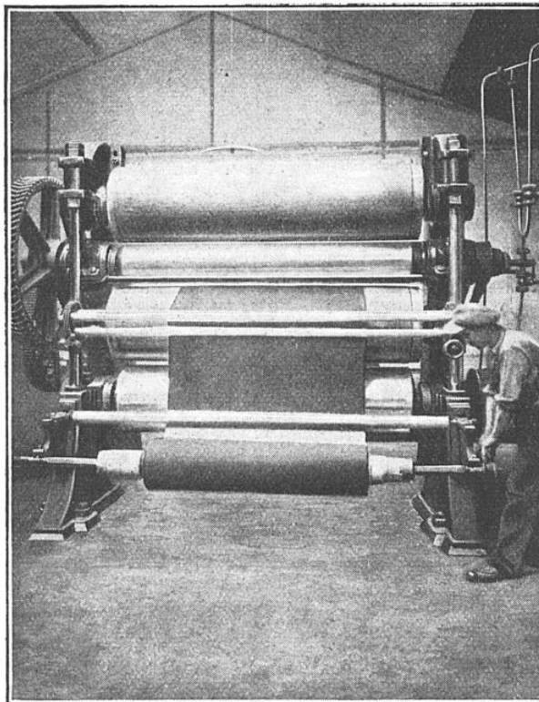
MACHINE A CYLINDRES, DITE « MAROQUINEUSE » Quand le caoutchoutage a pour but la production de cuirs factices (pour capotes de voitures, par exemple, ou pour l'ameublement), on passe le tissu entre des cylindres gravés qui lui donnent le grain du maroquin.
