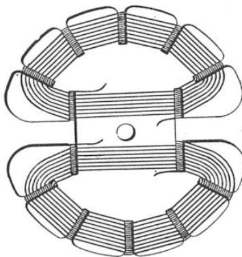
FIG. 2. — VARIOMÈTRE TYPE EN D
