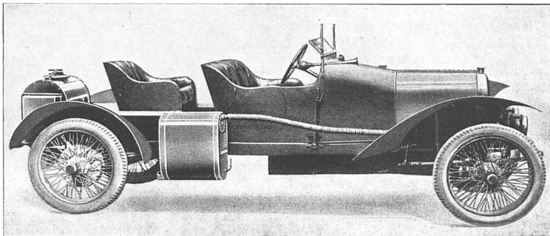
VOITURE DE TOURISME MUNIE D'UN GAZOGÈNE « AUTOGAZ »
