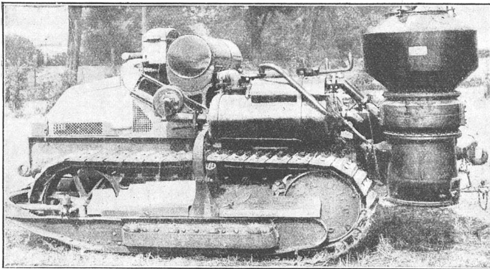
Le Gazogène ÉTIA alimentant le Tracteur à chenilles Renault à la Semaine de Motoculture d'Essonne
