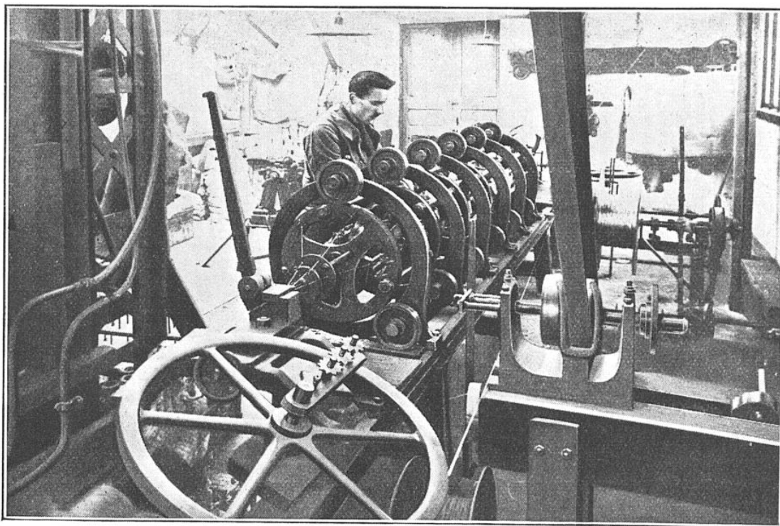
FIG. 10. — CABLEUSE A GRANDE VITESSE FOURNISSANT DU CÂBLE A SEPT FILS
