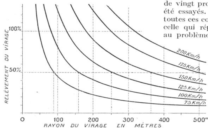
TRACÉ SCHÉMATIQUE DES RELÈVEMENTS D'UNE PISTE PAR RAPPORT AUX RAYONS
