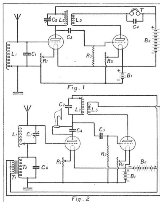
PLANCHE 2. — AUTRES TYPES DE POSTES A DEUX LAMPES
