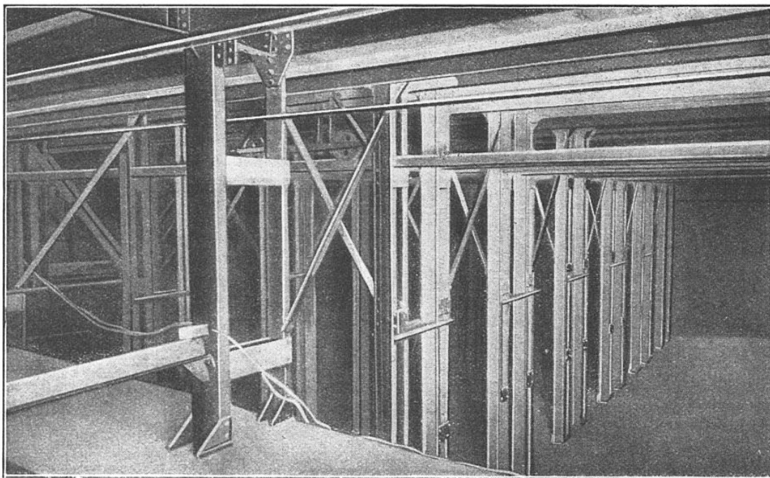
ENTRE CES NOMBREUX POINTS D'APPUI, LE PLANCHER DE SCÈNE EST MOBILE PAR SECTIONS
