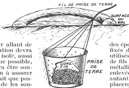
FIG. 2. — DISPOSITION DU RÉCIPENT À DEMI REMPLI DE COKE
