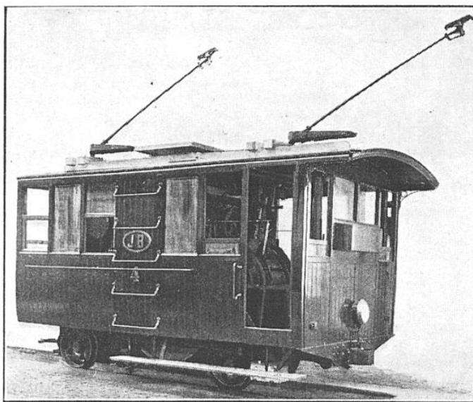
VUE EXTÉRIEURE DE LA LOCOMOTIVE A CRÉMAILLÈRE, ALIMENTÉE PAR DU COURANT TRIPHASÉ, DU CHEMIN DE FER DE LA JUNGFRAU
