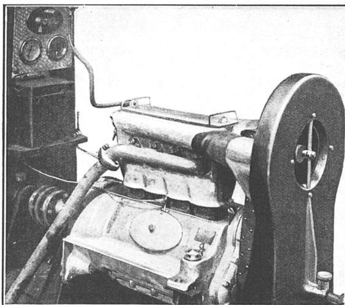
LE MOTEUR AU BANC D'ESSAI, COTÉ ÉCHAPPEMENT En avant est disposée la turbine de refoulement d'air, reliée aux tubulures et au carter de refroidissement.
