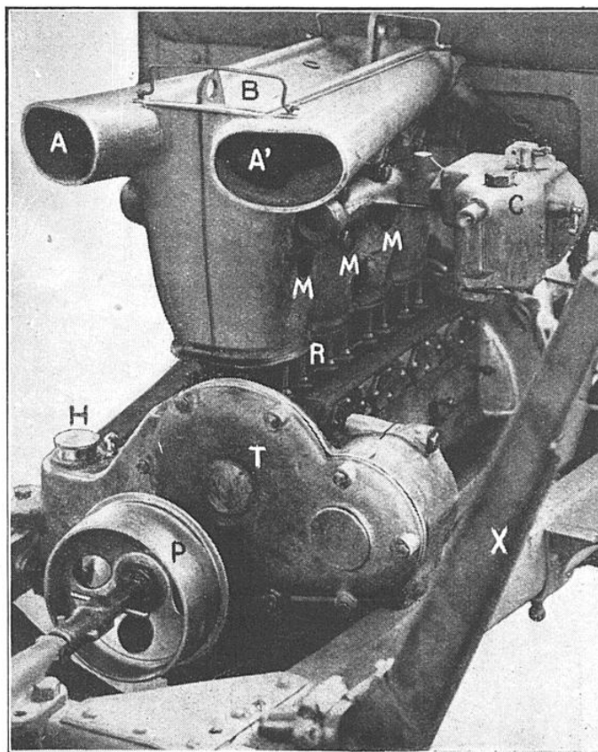
LE MOTEUR VU DE L'AVANT, LA FACE ENLEVÉE
