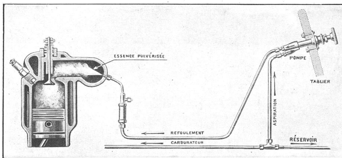
VUE SCHÉMATIQUE DU MODE DE MONTAGE DE L'INJECTEUR
