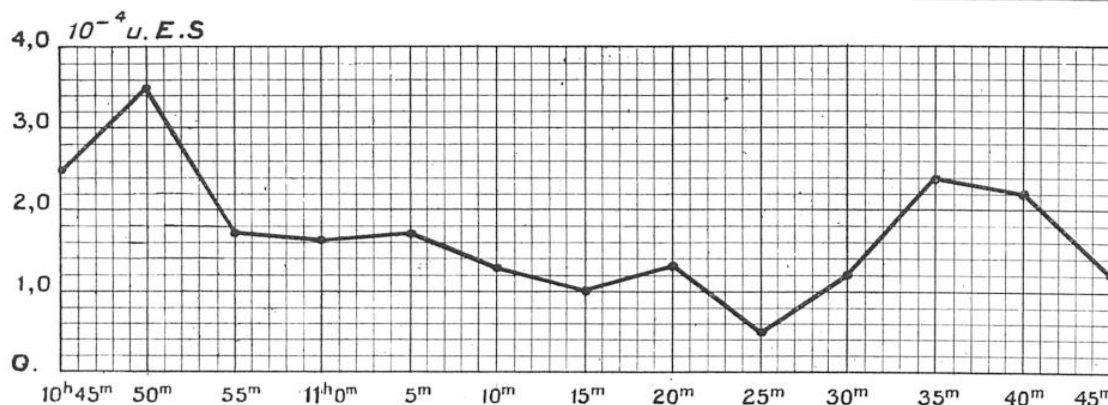
FIG. 4. — GRAPHIQUE DE L'ACTIVITÉ RELATIVE DE LA RADIATION SOLAIRE ULTRA-VIOLETTE. Ce graphique a été établi à Paris, le 4 novembre 1923, à l'aide de l'actinomètre photo-électrique du Dr Szilard. Les temps (en heures et minutes) sont portés en abscisses et les intensités correspondantes des radiations ultra-violettes (en unités électrostatiques) en ordonnées. L'allure de la courbe est due à l'absorption des radiations par le passage rapide de petits nuages à l'horizon.
