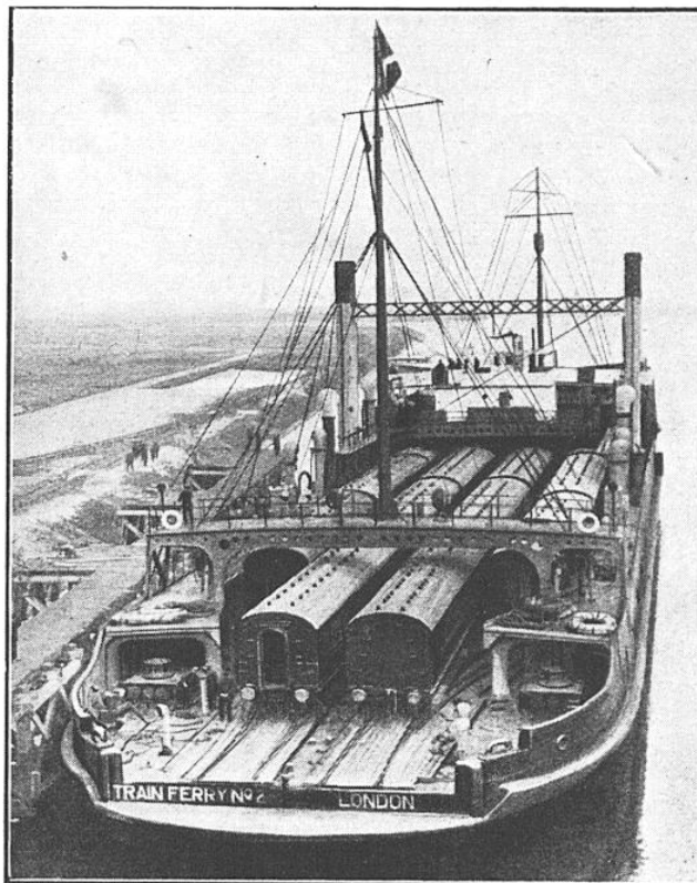
UN CHARGEMENT DE 18 VOITURES DE 28 TONNES ET 18 MÈTRES DE LONGUEUR CHACUNE
