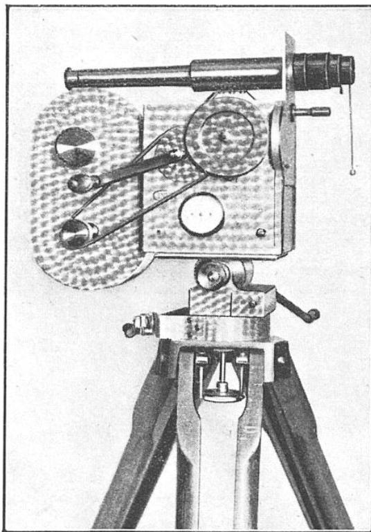
L'APPAREIL DE PRISE DE VUES, PROJECTION, TIRAGE ET AGRANDISSEMENT « CINEX »
