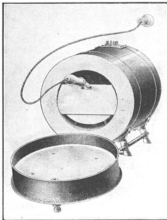
LE FOUR ÉLECTRIQUE « CLIN » AVEC L'APPAREIL A FAIRE DES GRILLADES
