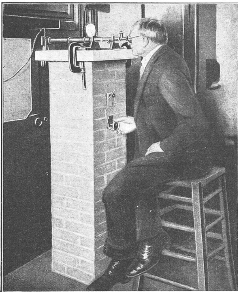
FIG. 2. — LES OPÉRATIONS DE MESURE DU POIDS DU CRISTAL S'EFFECTUENT DE L'EXTÉRIEUR, AU MOYEN DE TIGES DE MANŒUVRE. Cette précaution assure la constance de température nécessaire pour une pesée aussi délicate.
