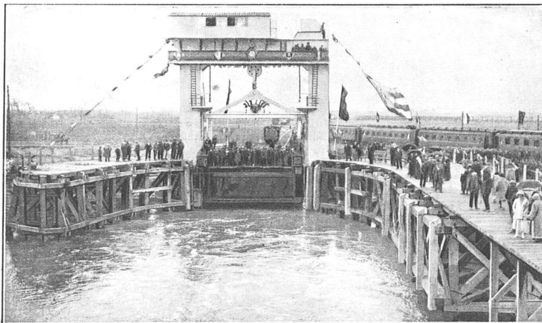
APPONTEMENT ET PASSERELLE INSTALLÉS A ZEEBRUGGE POUR LES FERRY-BOATS
