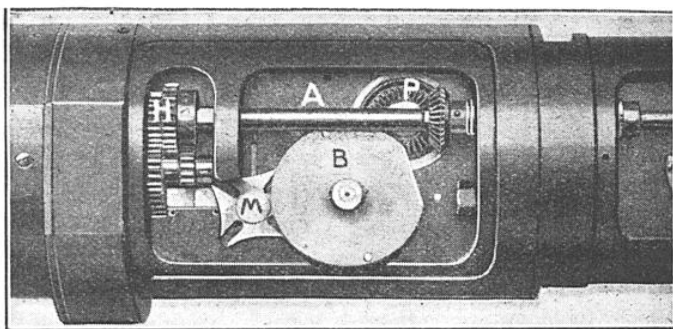
FIG. 6. — COMMANDE DU MÉCANISME DU CINÉMA
