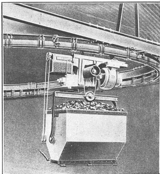
PALAN ÉLECTRIQUE COMBINÉ AVEC UN CHA- RIOT, SYSTÈME TOURTELLIER
