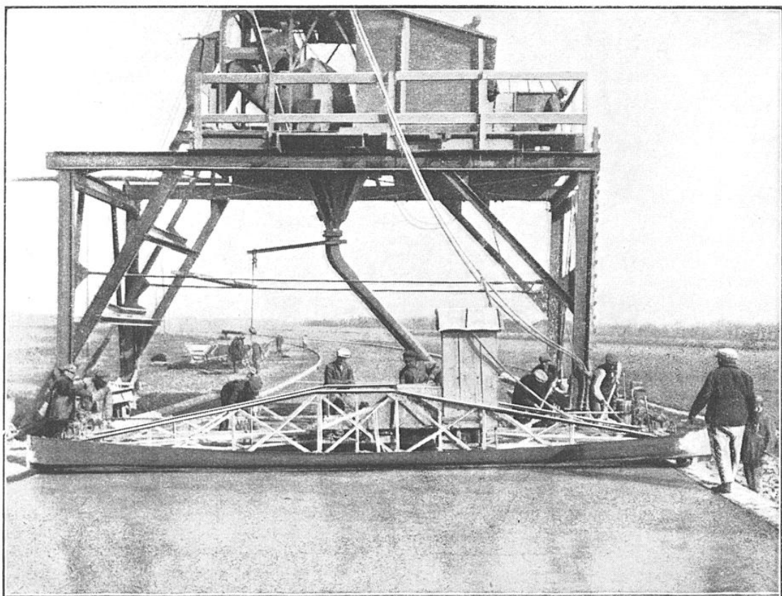
L'ÉPANDAGE MÉCANIQUE DU CIMENT SUR UNE PISTE AUTOMOBILE
