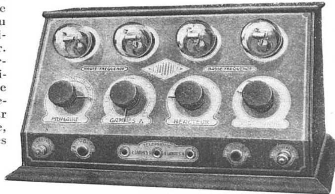
POSTE DE RÉCEPTION BELGE A QUATRE LAMPES, PERMETTANT LA RÉCEPTION DE TOUTES LES LONGUEURS D'ONDES ET L'AUDITION EN HAUT-PARLEUR
