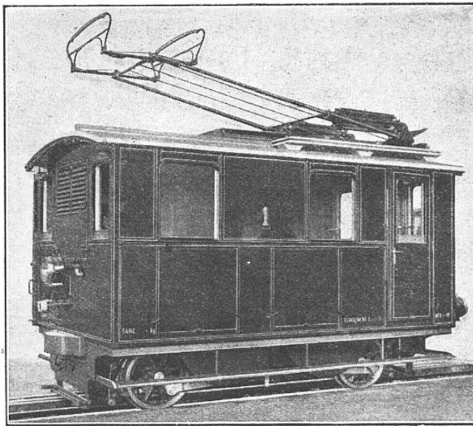
VUE EXTÉRIEURE DE LA LOCOMOTIVE DE LA LIGNE MIXTE BLONAY-LES-PLÉIADES (SUISSE)
