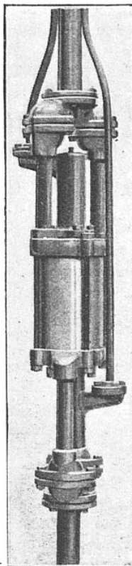
CORPS CYLINDRIQUE DE LA POMPE POUR PUITTS PROFONDS
