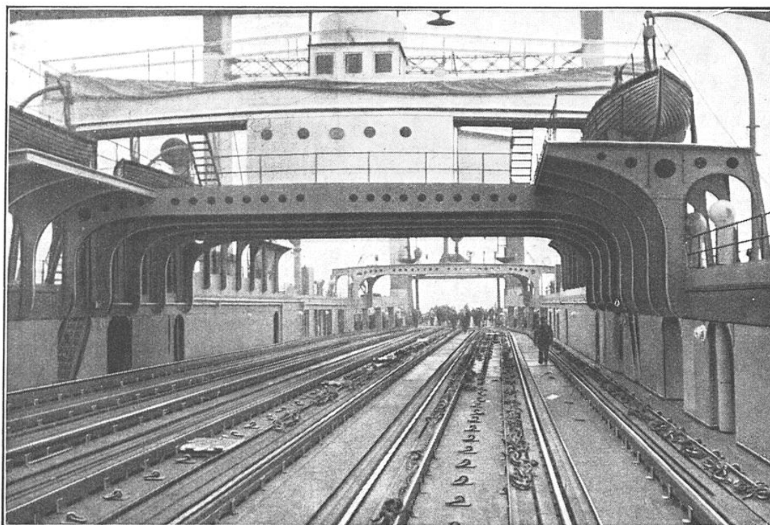
PHOTOGRAPHIE DE L'INTÉRIEUR D'UN FERRY-BOAT, AMARRÉ A L'APPONTEMENT ET RELIÉ AU RÉSEAU FERRÉ CONTINENTAL PAR LA PASSERELLE
