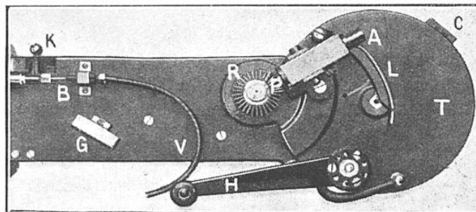
FIG. 2. — LA CROSSE DE L'HORO-CINÉ
