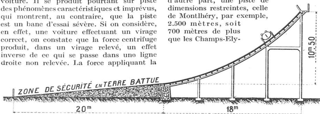
COUPE DE LA PISTE DE MONTLHÉRY DANS UN VIRAGE
