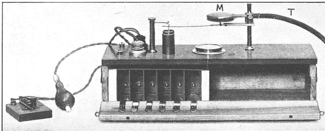
VUE D'ENSEMBLE DE LA BOÎTE A CONTACTS ÉLECTRO-PNEUMATIQUES
