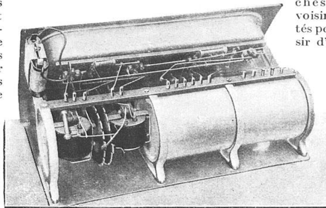
L'APPAREIL SORTI DE SON COFFRE ET VU PAR L'ARRIÈRE. Au premier plan, les trois cages de Faraday, dont l'une, ouverte, laisse voir les organes internes.
