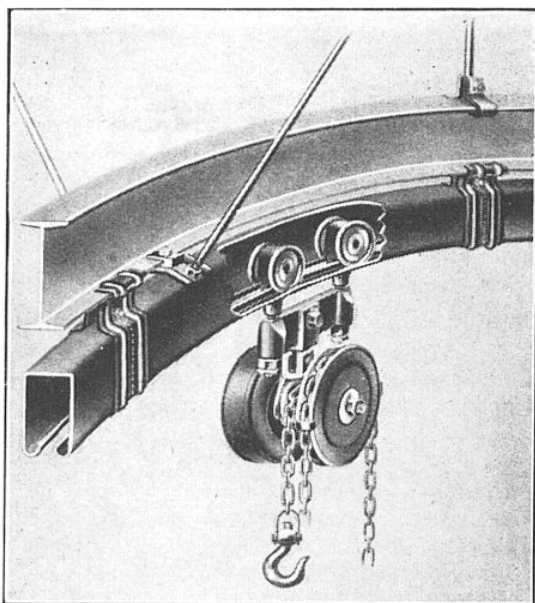
COUPE PARTIELLE MONTRANT LE ROULEMENT DES GALETS DANS LE RAIL
