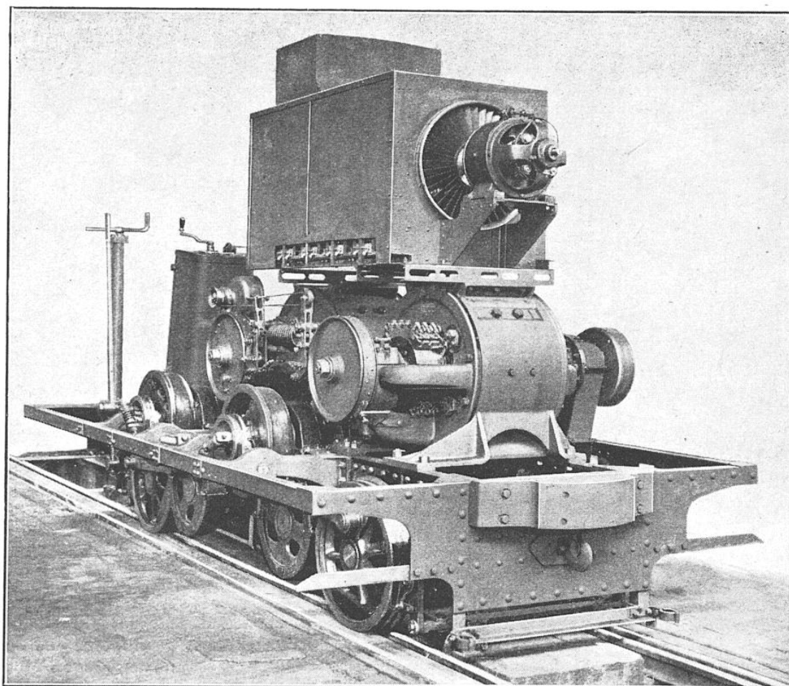
ENSEMBLE DES ORGANES DE LA LOCOMOTIVE DE LA LIGNE MIXTE BLONAY-LES-PLÉIADES, PRÈS DE VEVAY (SUISSE)
