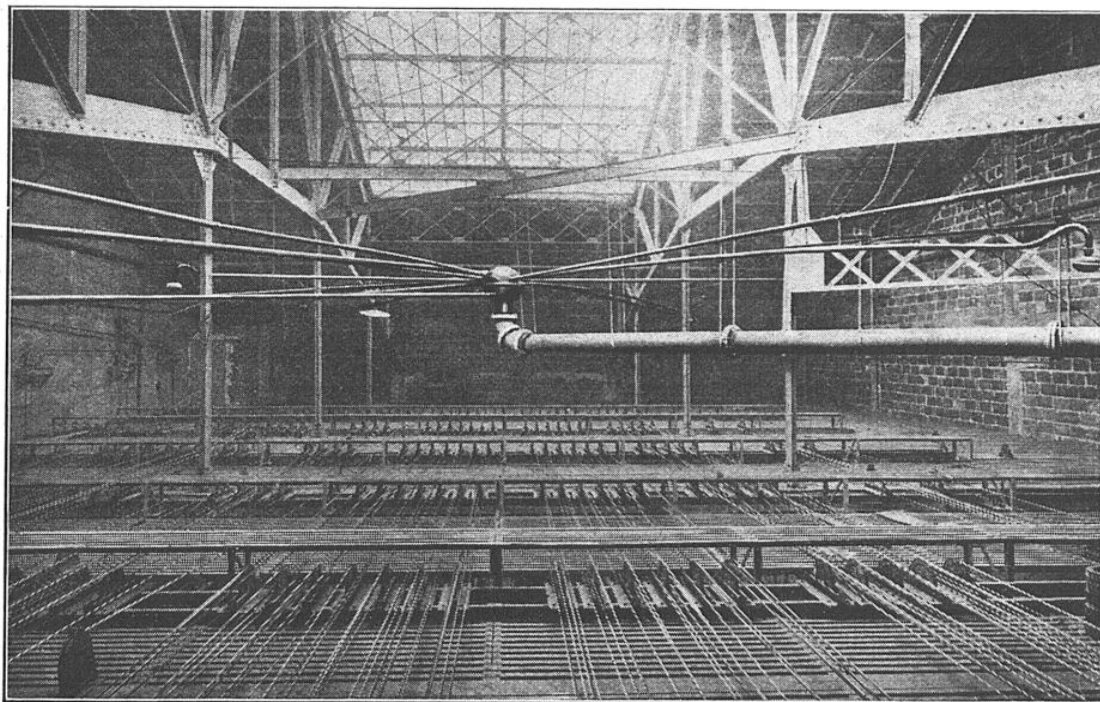
L'INSTALLATION DU « GRAND SECOURS » CONTRE L'INCENDIE AU-DESSUS DU GRIL
