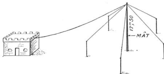
POSTE DE FORTUNE DE LA STATION D'ABADLA, CERCLE DE COLOMB-BÉCHAR
