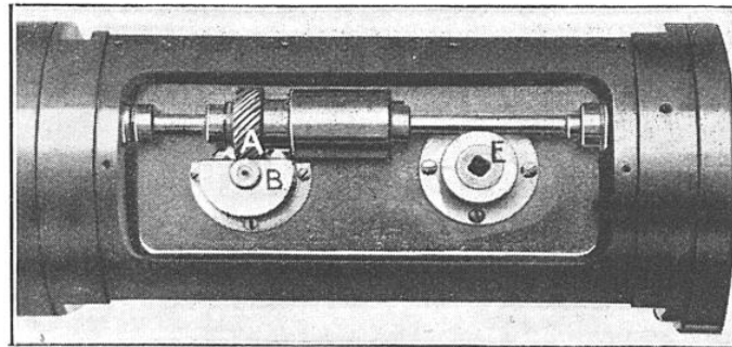
FIG. 4. — VUE DES ORGANES DE COMMANDE DE LA BOÎTE-MAGASIN
