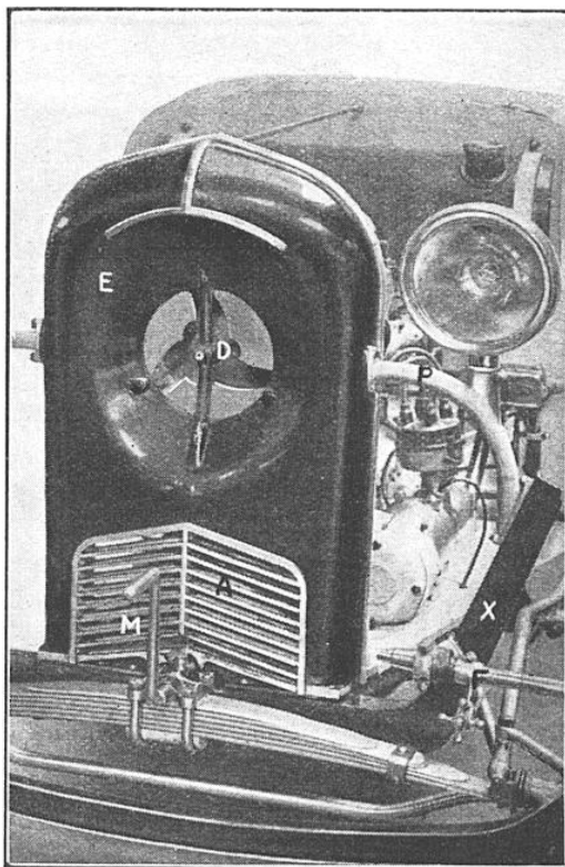
FAÇADE DU CHASSIS « SARA »
