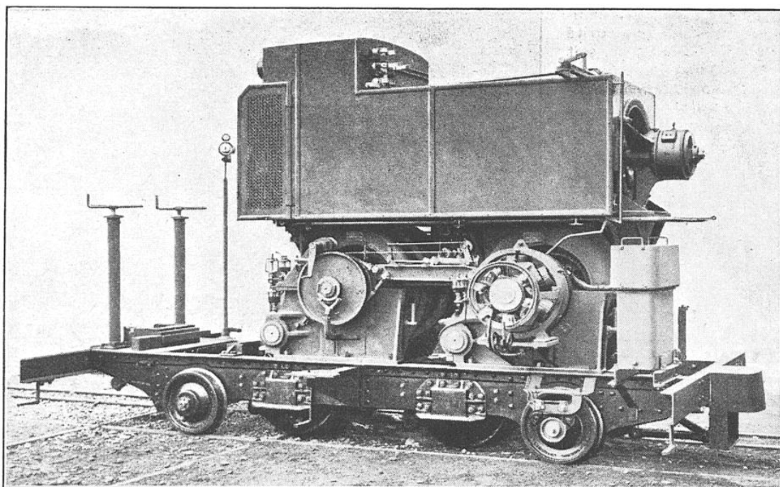
ORGANES INTÉRIEURS DE LA LOCOMOTIVE DE LA LIGNE DE RIO-DE-JANEIRO
