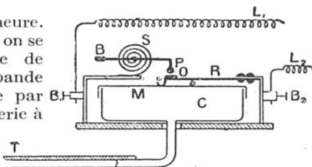
SCHÉMA DE LA CAPSULE MAREY
