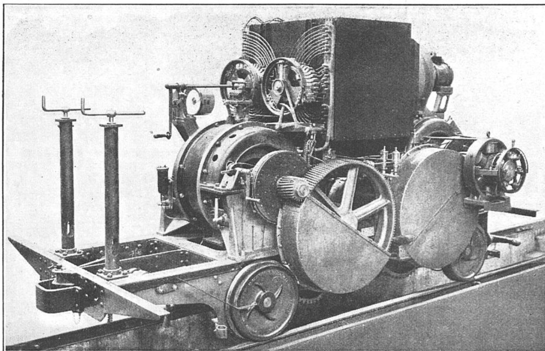
LA MACHINE FIGURÉE A LA PAGE PRÉCÉDENTE AVEC SON ARMATURE ENLEVÉE
