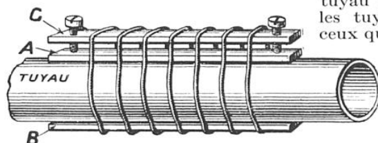
FIG. 1. — MANIÈRE D'AMÉNAGER UNE CANALISATION D'EAU POUR SERVIR DE PRISE DE TERRE EXCELLENTE
