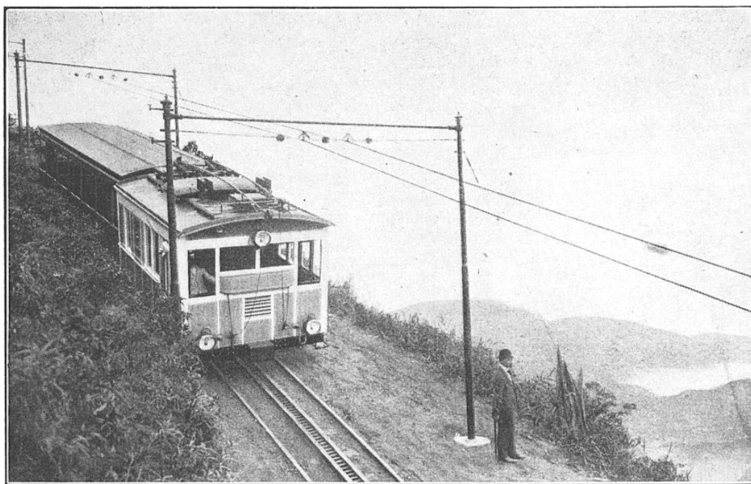
TRAIN DESCENDANT UNE VOIE A CRÉMAILLÈRE SYSTÈME RIGGENBACH
