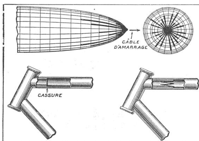
CETTE FIGURE MONTRÉ LE PRINCIPE DE LA RÉPARTITION DE L'EFFORT, QUI EST LE MÊME APPLIQUÉ À LA FABRICATION D'UN CADRE DE BICYCLETTE ET À LA FIXATION DU CÂBLE D'AMARRAGE SUR LA CARCASSE D'UN AÉRONEF
