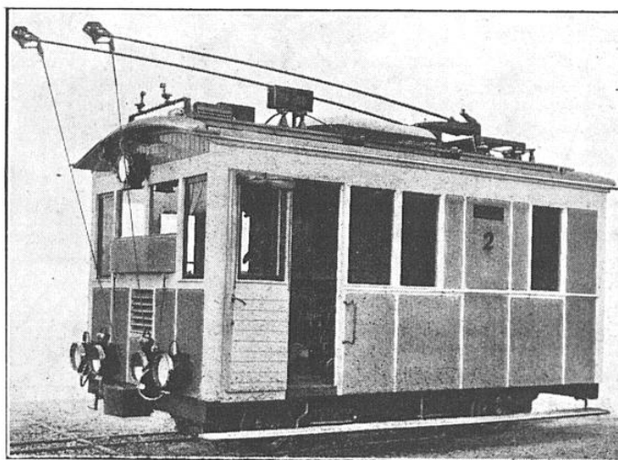
VUE EXTÉRIEURE DE LA LOCOMOTIVE DE LA LIGNE DE RIO-DE-JANEIRO A CORCOVADO
