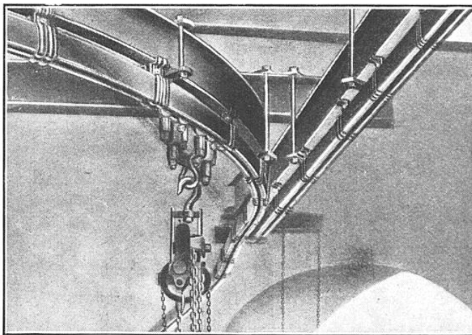
AIGUILLAGE A PIVOT
