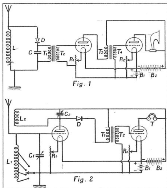
PLANCHE 1. — CIRCUITS A GALÈNE ET A LAMPES COMBINÉES
