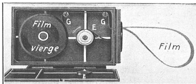
FIG. 3. — VUE DE LA BOITE-MAGASIN
