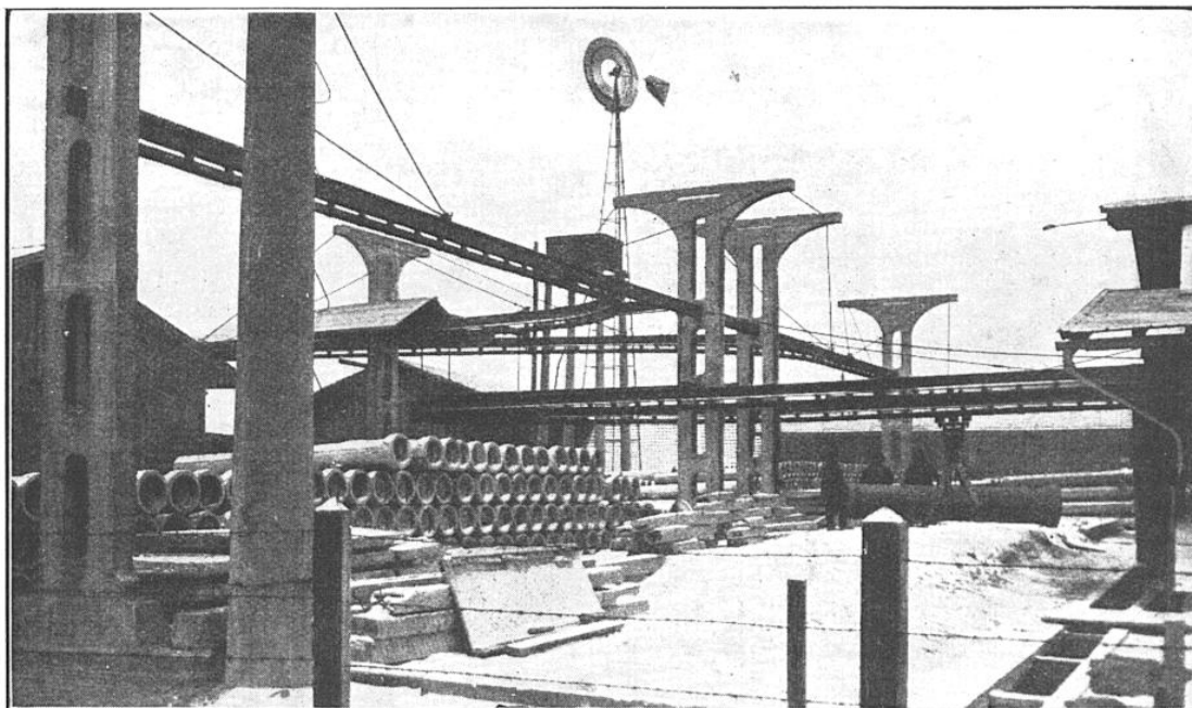
LA NEIGE NE GÊNE NULLEMENT LES MANUTENTIONS PAR VOIE SUSPENDUE
