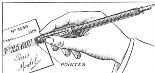
L'EXTRÉMITÉ, MUNIE DE POINTES DU STYLOGRAPHE, RAYE LE PAPIER ET EMBLIT D'ENCRE INDÉLÉBILE LES SILLONS TRACÉS.
