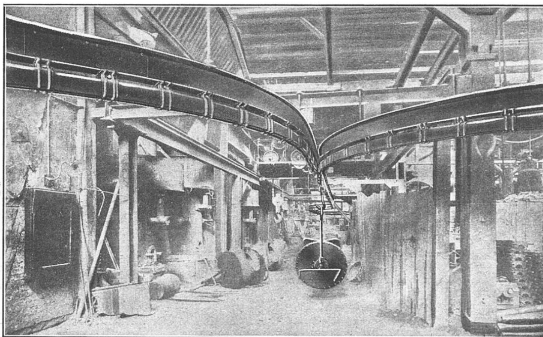
INSTALLATION D'UN TRANSPORTEUR MONORAIL DANS UNE FONDERIE
