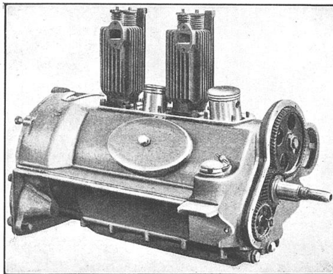
MOTEUR DÉPOUILLÉ DU CARTER DE REFROIDISSEMENT Deux cylindres sont en place, laissant voir la disposition de leurs ailettes verticales de refroidissement.
