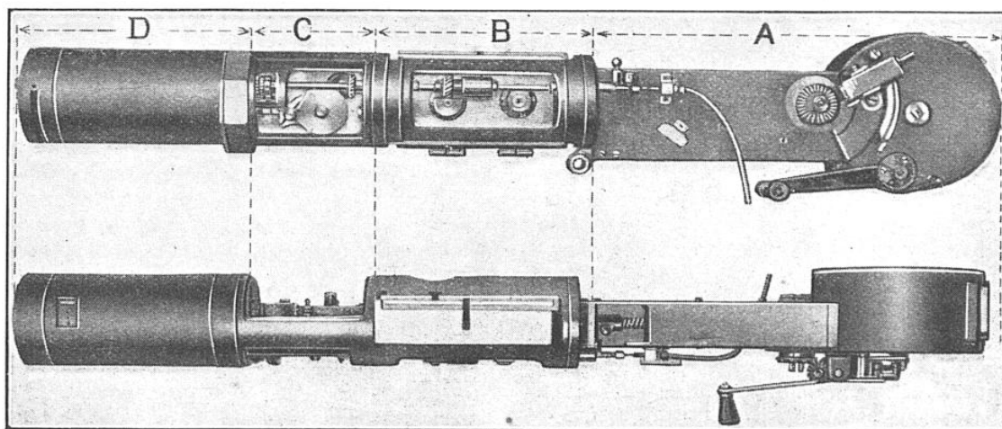
FIG. 1. — L'HORO-CINÉ VU DE COTÉ (EN HAUT), VU EN PLAN (EN BAS) A , crosse de l'appareil ; B , support de la boîte-magasin ; C , mécanisme ; D , logement de la partie optique.
