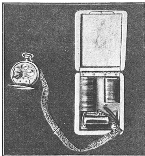
DISPOSITIF DE REMISE A L'HEURE D'UNE MONTRE PAR T. S. F.
