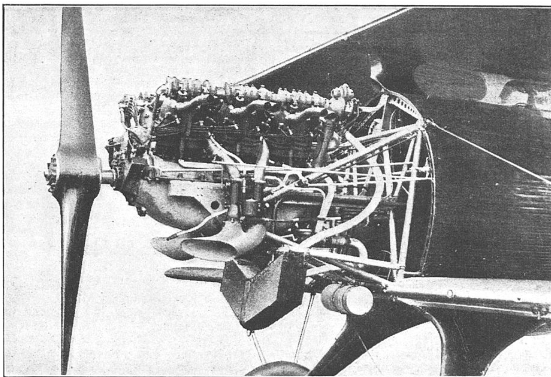
MOTEUR DE 400 CHEVAUX, MIS EN PLACE SUR L'AVION, AVEC LEQUEL PELLETIER DOISY A EFFECTUÉ LE VOYAGE DE PARIS AU TONKIN
