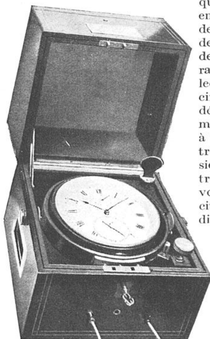
CHRONOMÈTRE A CONTACTS ÉLECTRIQUES
