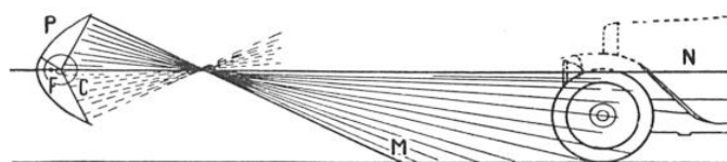
INDICATION SCHÉMATIQUE DU DEMI-ÉCLAIRAGE
