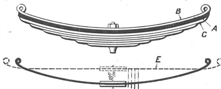
FIGURES MONTRANT LA DÉFORMATION D'UN RESSORT A, lame-frein; B, C, lames maîtresses du ressort; E, position du ressort sous une flèche de 10 centimètres.
