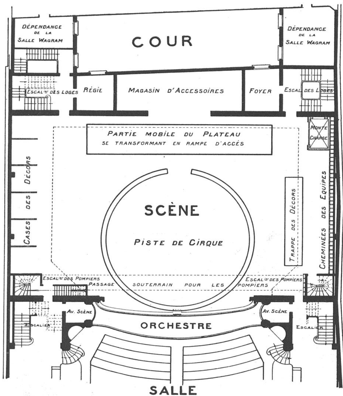
PLAN DE LA SCÈNE ET DE SES ANNEXES AU NIVEAU DU PLATEAU
