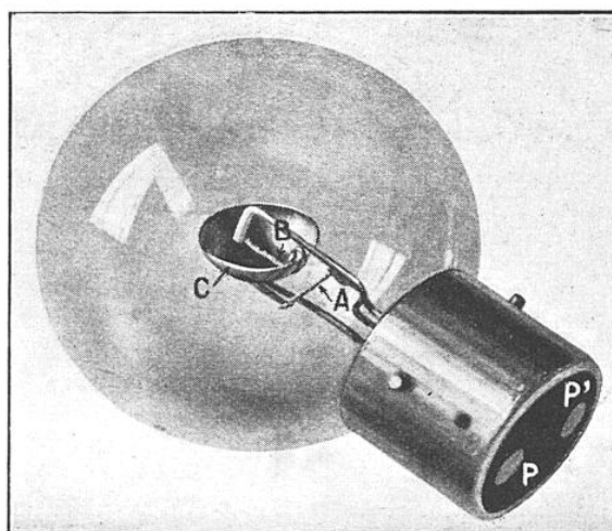
L'AMPOULE A DOUBLE FILAMENT
