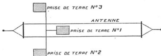
FIG. 3. — LES PRISES DE TERRE INSTALLÉES EN TRIANGLE
