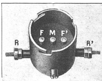
DÉTAIL DE LA DOUILLE A TROIS CONTACTS
