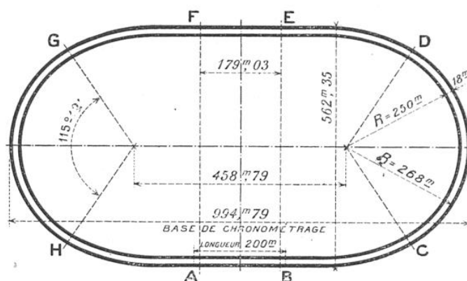
PLAN DE LA PISTE PARISIENNE DE MONTLHÉRY
