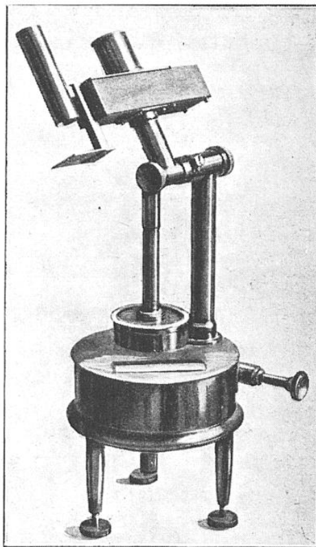
FIG. 2. — VUE AGRANDIE DE L'ACTINOMÈTRE SOLAIRE PHOTO-ÉLECTRIQUE L'appareil se compose d'une cellule photo-électrique en quartz (très sensible), à cathode en cadmium, servant de détecteur, et d'un électromètre à cadran dont le déplacement de l'aiguille mesure l'intensité des radiations ultra-violettes. (Voir fig. 3 le dispositif intérieur de l'appareil.)
