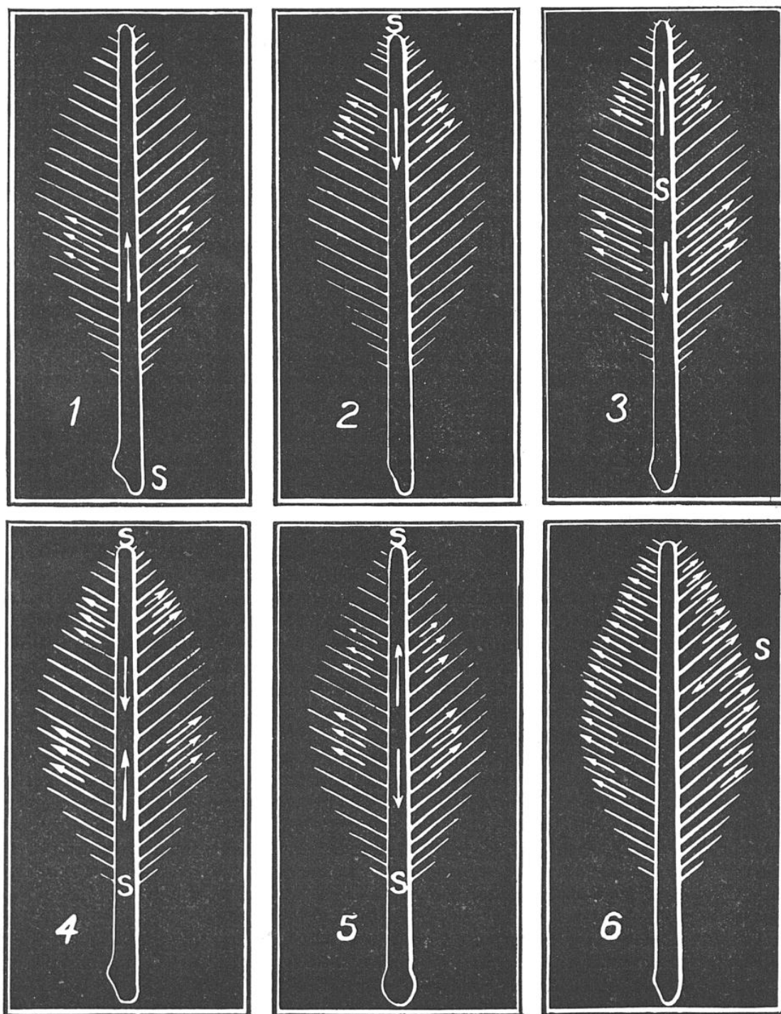
PLUMES DE MER SCHÉMATISÉES. — Les flèches indiquent le sens de la propagation de l'onde photogène, vraisemblablement accompagnée d'une onde électromotrice. — La lettre S placée en divers endroits des figures montre le point excité.
