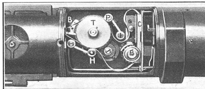
FIG. 5. — MÉCANISME DU CINÉMA
