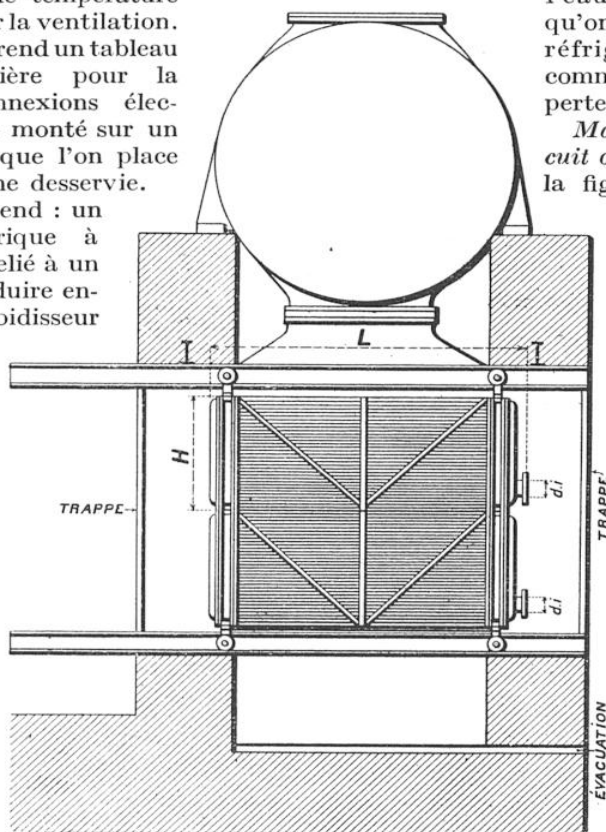
FIG. 2. — COUPE DE LA CHAMBRE DU REFROIDISSEUR D'AIR (SYSTÈME SCAM-VICKERS)
