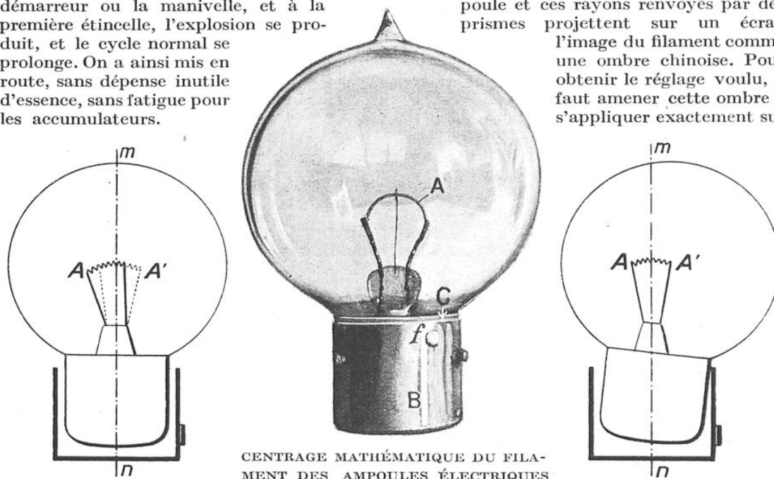
Au milieu, vue extérieure de la lampe. A, filament électrique ; B, culot ; C, douille solidaire de l'ampoule ; f, point de soudure. A gauche et à droite, coupe schématique de la lampe. A, mauvaise position du filament ; A', bonne position. Après réglage, A et A' se confondent.
