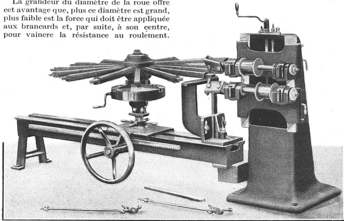
MACHINE A FAIRE LES BROCHES OU TENONS DES RAIS DE ROUES S'ENGAGEANT DANS LES JANTES (DIAMÈTRE MAXIMUM DES ROUES : 3 M. 20)
