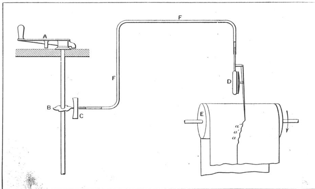
FIG. 5. — DISPOSITIF MÉCANIQUE ET PNEUMATIQUE DE TRANSMISSION ET ENREGISTREMENT DES MANŒUVRES EXÉCUTÉES PAR LE CANDIDAT WATTMAN
