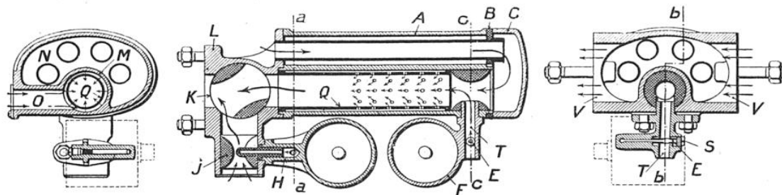
DIVERSES COUPES DU CARBURATEUR A HUILES LOURDES
