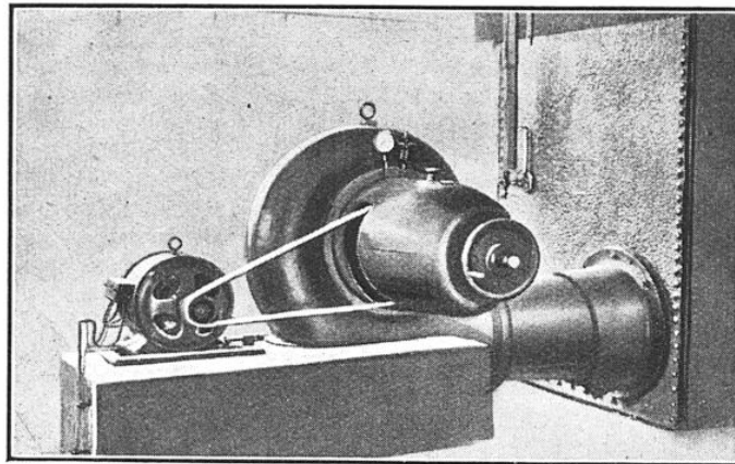
FIG. 6 — VUE D'UNE TURBINE AUTORÉGULATRICE ASSURANT L'ÉCLAIRAGE ET LE CHAUFFAGE D'UNE MAISON PARTICULIÈRE
