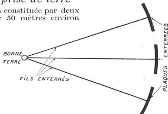
SCHÉMA D'UNE BONNE PRISE DE TERRE
