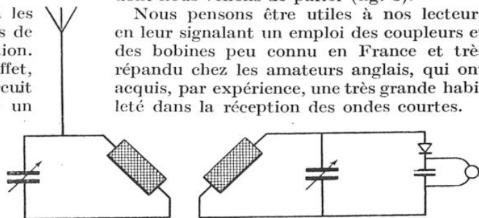
FIG. 2. — SCHÉMA D'UN CIRCUIT CONSTITUÉ PAR DEUX BOBINES « NID D'ABEILLE »
