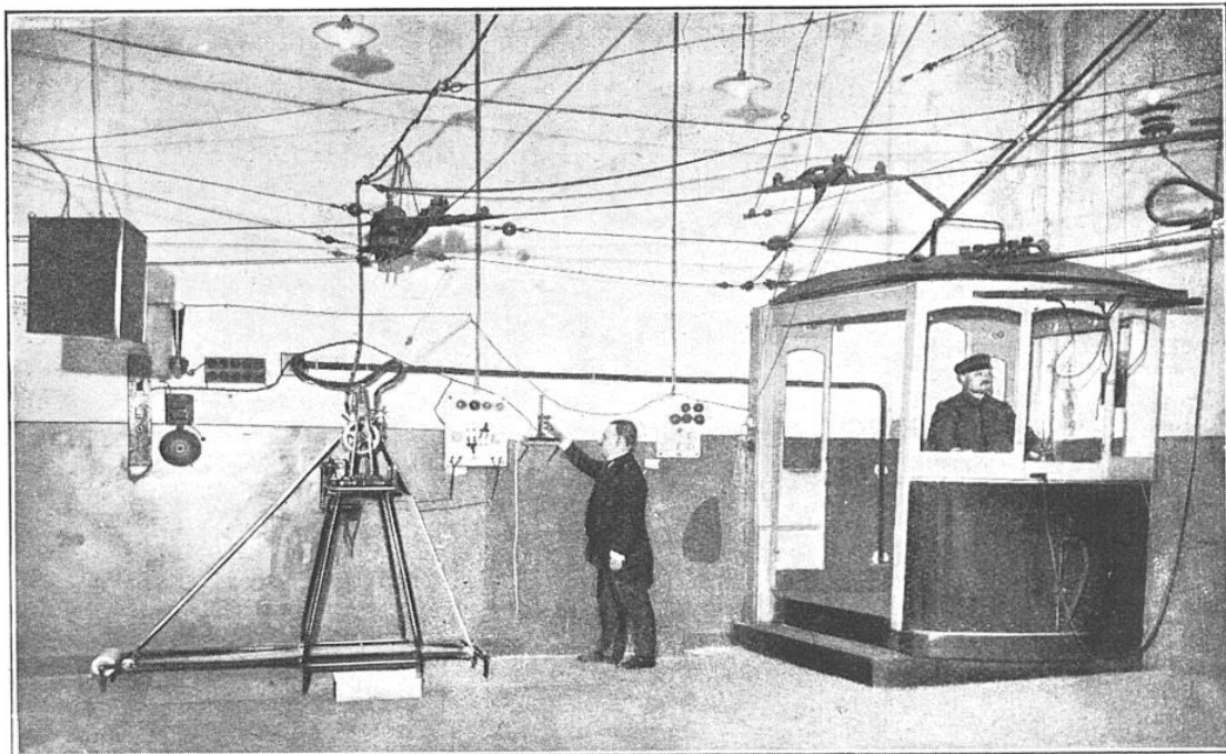
FIG. 1. - VUE D'ENSEMBLE DE L'INSTALLATION PSYCHOTECHNIQUE DES TRAMWAYS BRUXELLOIS On aperçoit, à droite de la photographie, l'avant du tramway où prend place le candidat à examiner et, à gauche, l'appareil enregistreur. De-ci de-là sont répartis dans la salle divers signaux sonores et lumineux, qui, pour le candidat, sont autant de prétextes à bien ou mal manœuvrer.
