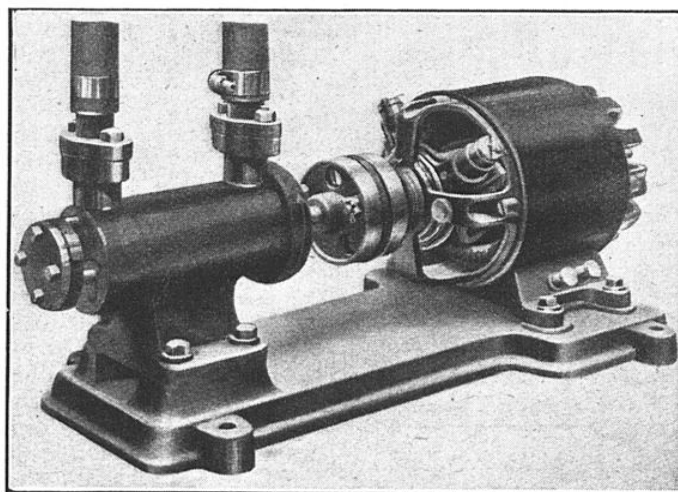
VUE D'ENSEMBLE DE LA POMPE S.A.M. ET DE SON MOTEUR
