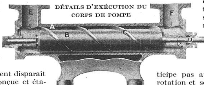
A, corps cylindrique ; B, tambour ; C, filets hélicoïdaux ; D, axe relié au moteur ; EF, brides d'admission et de refoulement.
