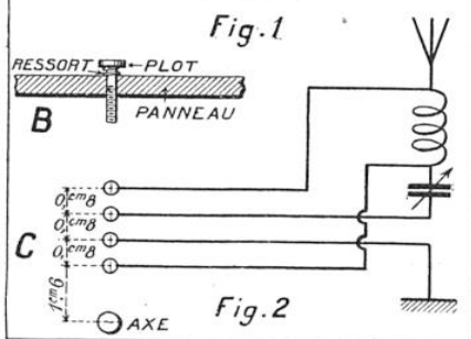
DISPOSITIF DU COMMUTATEUR SÉRIE-PARALLÈLE
