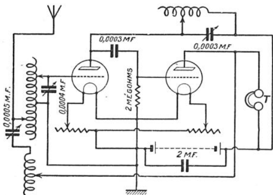
FIG. 2. — MONTAGE REINARTZ AVEC AMPLIFICATEUR H. F. ET ANODE ACCORDÉE
