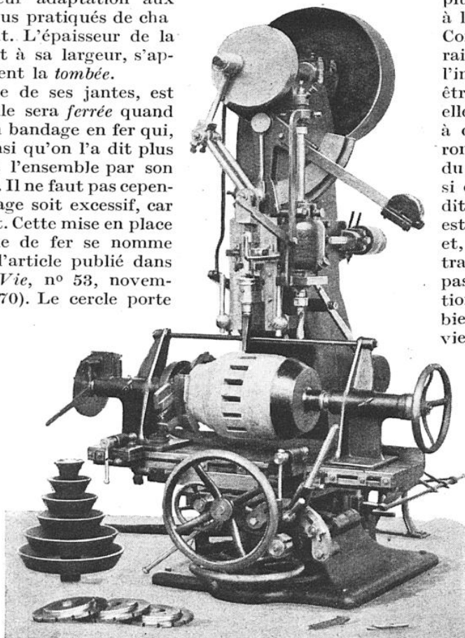
GRANDE MACHINE A MORTAISER LES MOYEUX JUSQU'À 550 MILLIMÈTRES DE DIAMÈTRE ET AUTANT DE LONGUEUR
