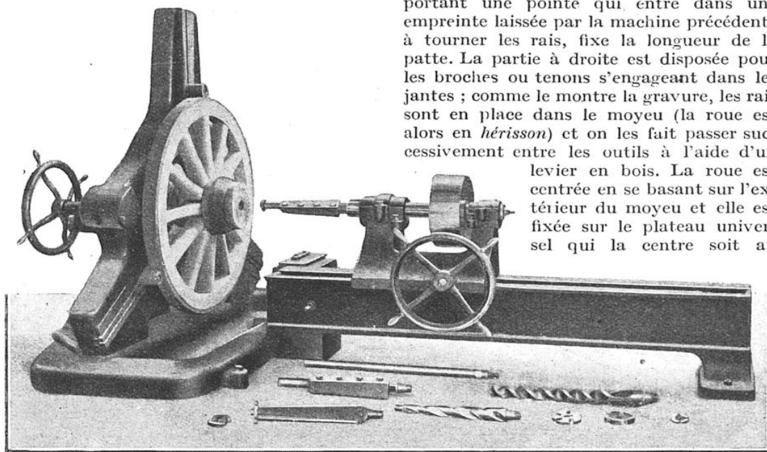
VUE D'ENSEMBLE D'UNE MACHINE À PERCER ET À ALÉSER LES MOYEURS DE ROUES JUSQU'À UN DIAMÈTRE MAXIMUM DE 2 MÈTRES
