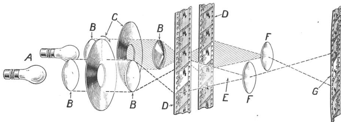
FIG. 3. — SCHÉMA DE LA PROJECTION DES DEUX FILMS EN FILM UNIQUE A EFFETS STÉRÉOSCOPIQUES (PRESSE DE TIRAGE PAR PULSATIONS)
