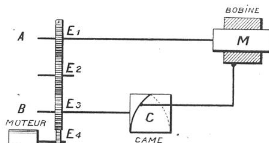
FIG. 5. — DESSIN SCHÉMATIQUE MONTRANT LE FONCTIONNEMENT DE LA MACHINE A FAIRE LES BOBINES « NID D'ABEILLE »
