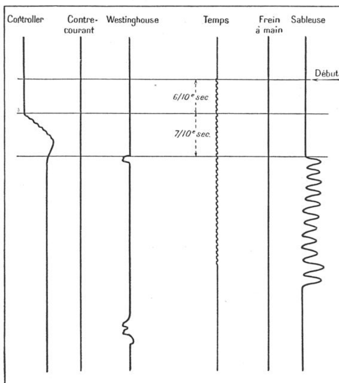
FIG. 6. — DIAGRAMMES DES TRACÉS CORRESPONDANT À UNE MANŒUVRE D'ARRÊT RAPIDE DU TRAMWAY
