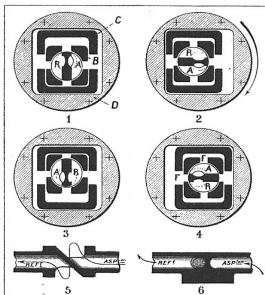
DIVERSES PHASES DU FONCTIONNEMENT DE LA POMPE SANS SOUPE
