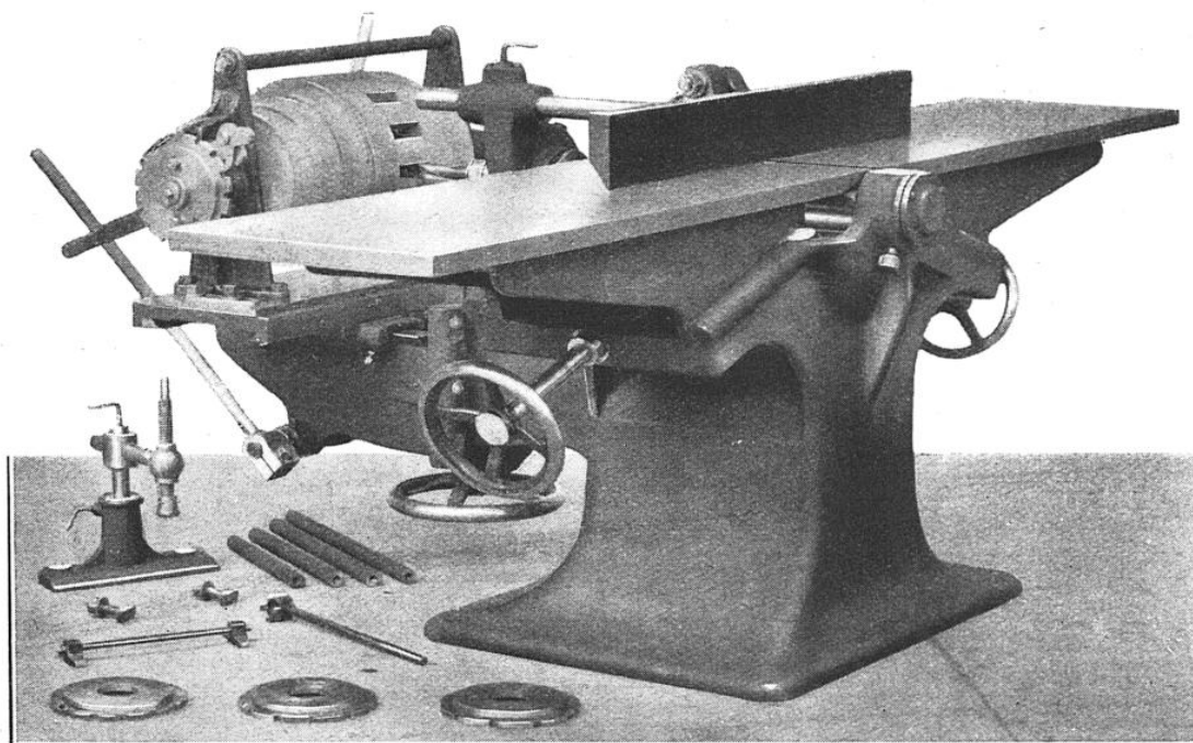
MACHINE COMBINÉE A DÉGAUCHIR, MORTAISER ET PERCER, AVEC APPAREIL A MORTAISER LES MOYEURS JUSQU'À 380 MILLIMÈTRES DE DIAMÈTRE
