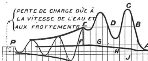
FIG. 2. — ESSAIS DE RENDEMENT DE LA SUPERTURBINE (MÉTHODE GIBSON)
