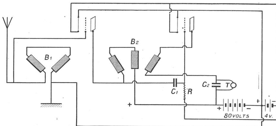
FIG. 4. — SCHÉMA D'UN MONTAGE TRÈS RÉPANDU PARMI LES AMATEURS ANGLAIS
