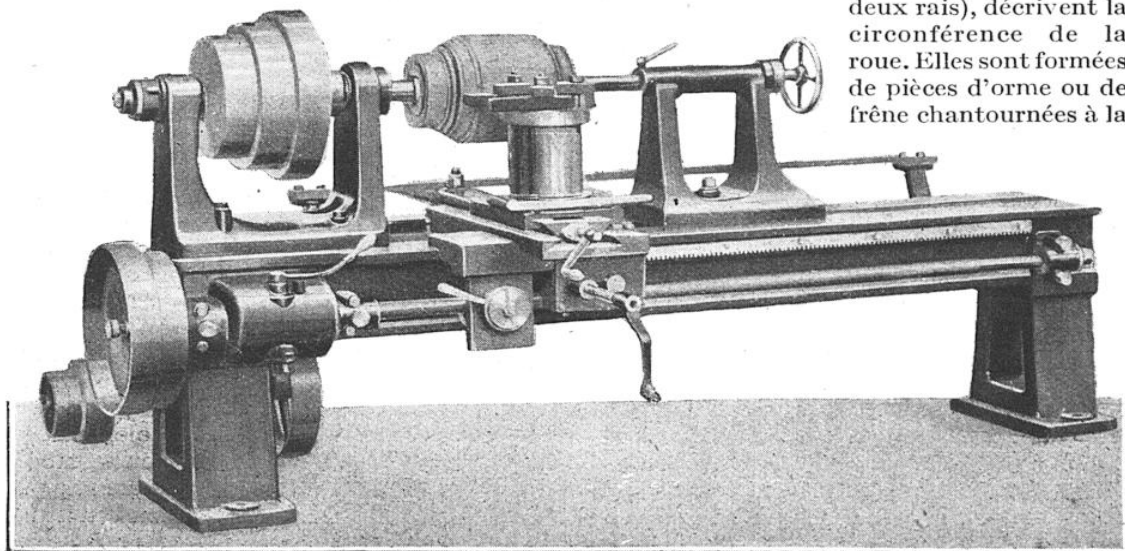
TOUR A TOUCHE POUR LA FABRICATION DES MOYEURS D'UN DIAMÈTRE MAXIMUM DE 550 MM.
