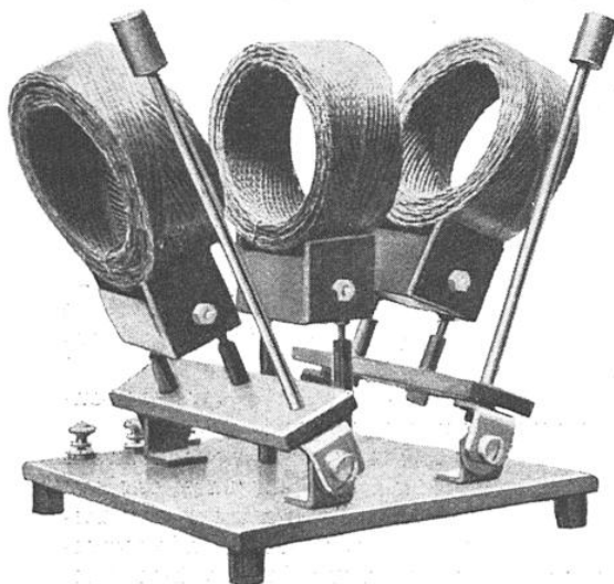
FIG. 3. — UN COUPLEUR A TROIS BOBINES « NID D'ABEILLE »
