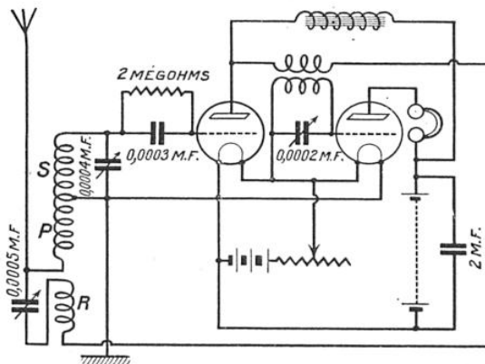
FIG. 3. — MONTAGE REINARTZ AVEC AMPLIFICATEUR H. F. ET TRANSFORMATEUR
