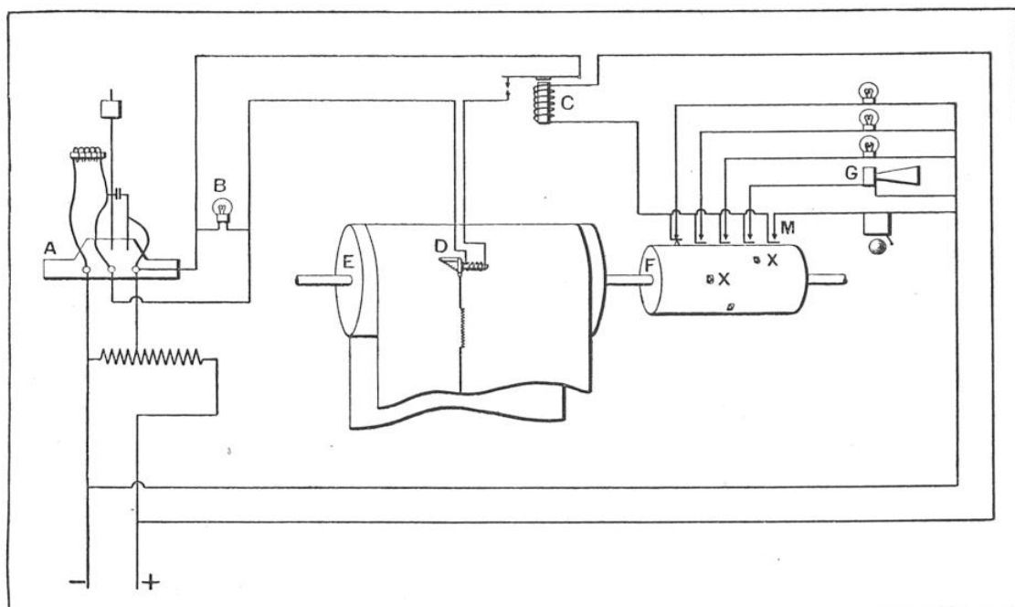
FIG. 3. — SCHÉMA DU DISPOSITIF ÉLECTROMÉCANIQUE D'ENREGISTREMENT D'UN SIGNAL ET, A DROITE, CYLINDRE DE MANŒUVRE DES CONTACTS RÉGLANT L'APPARITION DES SIGNAUX A, métronome à contact électrique, battant le dixième de seconde et permettant de lire l'enregistrement du signal en fonction du temps ; D, dispositif électromagnétique d'enregistrement ; E, cylindre enregistreur ; F, cylindre interrupteur ; G, signal ; M, contacts ; X X, crêtes du cylindre F.
