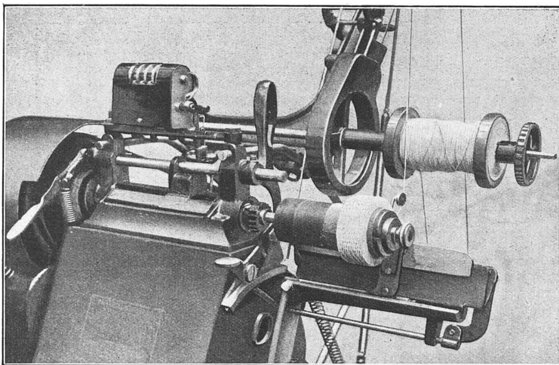
FIG. 6. — DÉTAILS DU MÉCANISME DE LA MACHINE A FABRIQUER LES BOBINES « NID D'ABEILLE » (VOIR L'ENSEMBLE FIG. 1)
