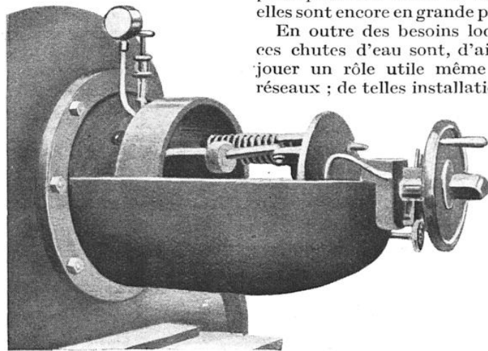
FIG. 5. — VUE DU VOLANT ET DU RÉGULATEUR CENTRIFUGE, LA PARTIE SUPÉRIEURE ENLEVÉE
