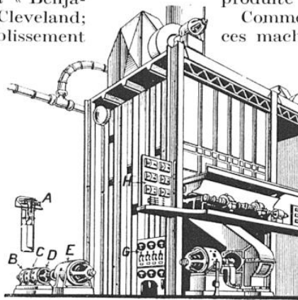
INSTALLATION COMPORTANT LE CONTROLE ÉLECTRIQUE DES FOYERS
