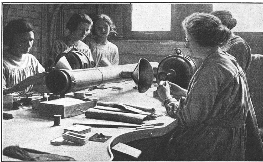
CONDUITS ET EMBOUCHURES D'ASPIRATION DANS UN ATELIER DE POLISSAGE OR ET PLATINE
