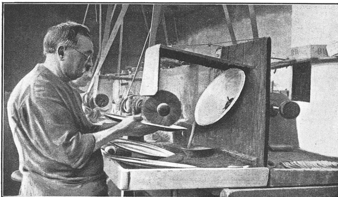
COMME POUR L'OR ET LE PLATINE, LE POLISSAGE DES PIÈCES EN ARGENT S'EFFECTUE ÉGALEMENT DEVANT L'ENTONNOIR D'UN CONDUIT D'ASPIRATION
