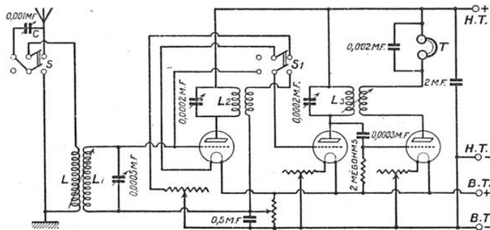
SCHÉMA DU NOUVEAU RÉCEPTEUR A TROIS LAMPES
