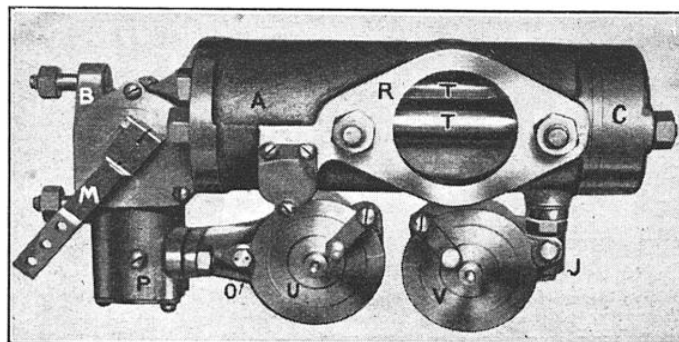
LE CARBURATEUR VU PAR DESSOUS
