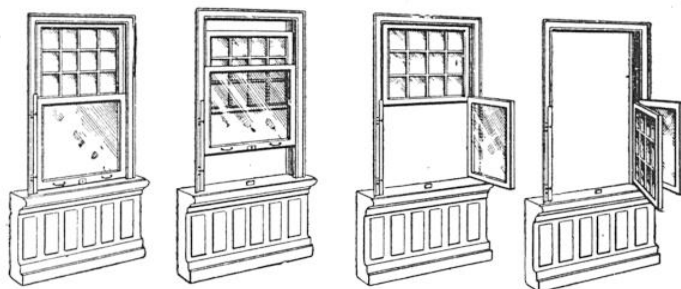
LES DEUX CHÂSSIS DE CETTE FENÊTRE À GUILLOTINE S'OUVRENT ET DÉMASQUENT ENTIÈREMENT L'OUVERTURE
