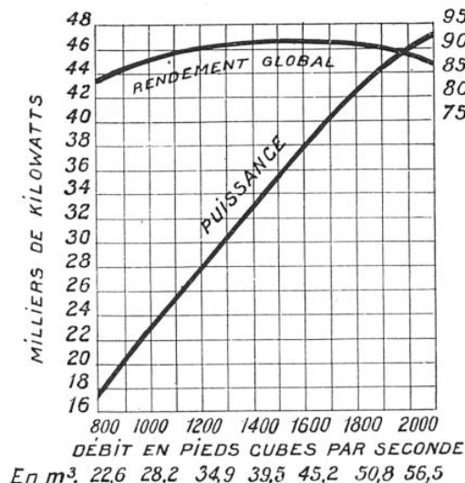
FIG. 3. — COURBES DE LA PUISSANCE ET DU RENDEMENT TOTAL DE LA SUPERTURBINE. Sur ce diagramme, les débits en pieds ou en mètres cubes par seconde sont portés en abscisses et les kilowatts obtenus (par milliers) sont portés en ordonnées. C'est le rendement global d'un groupe et de la puissance disponible aux bornes de l'alternateur en fonction de la quantité d'eau débitée par les conduites que ces deux courbes indiquent.
