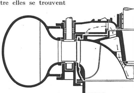
FIG. 1. — COUPE D'UNE SUPERTURBINE A TUBE D'ASPIRATION TRONÇONIQUE MOODY, DE 55.000 CHEVAUX
