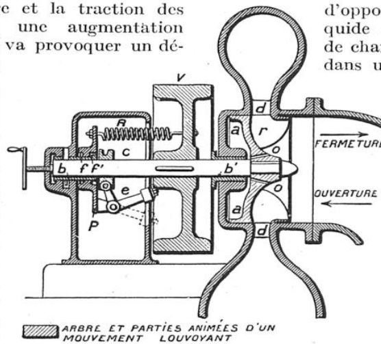
FIG. 4. — COUPE DE LA TURBINE AUTORÉGULATRICE ET DE SON MÉCANISME A MOUVEMENT LOUVOYANT
