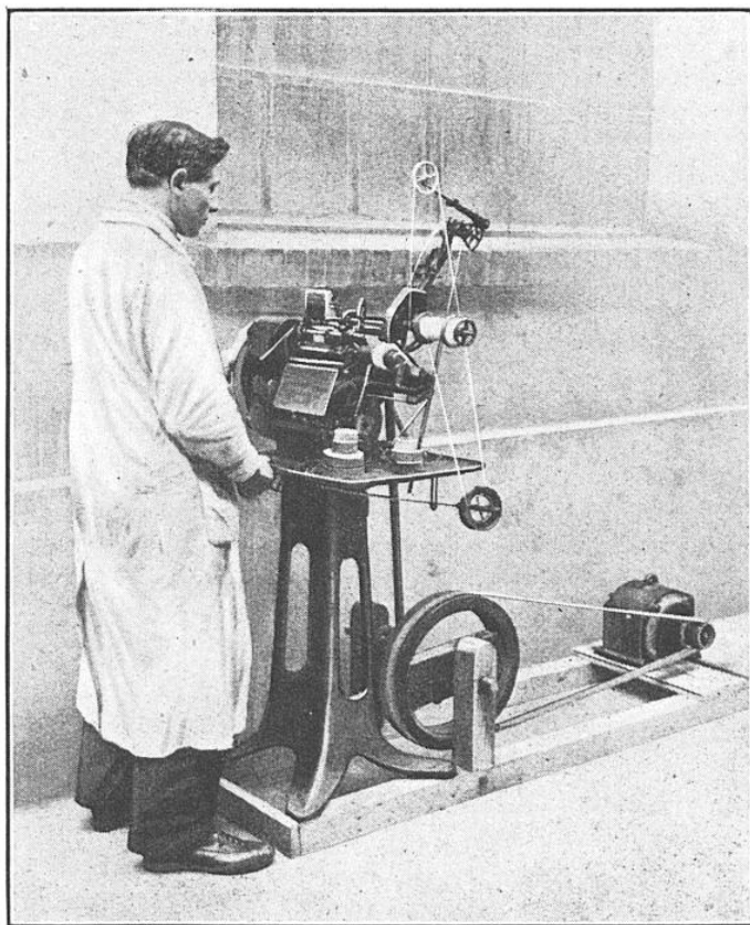
FIG. 1. — MACHINE A FABRIQUER LES BOBINES DITES « NID D'ABEILLE »
