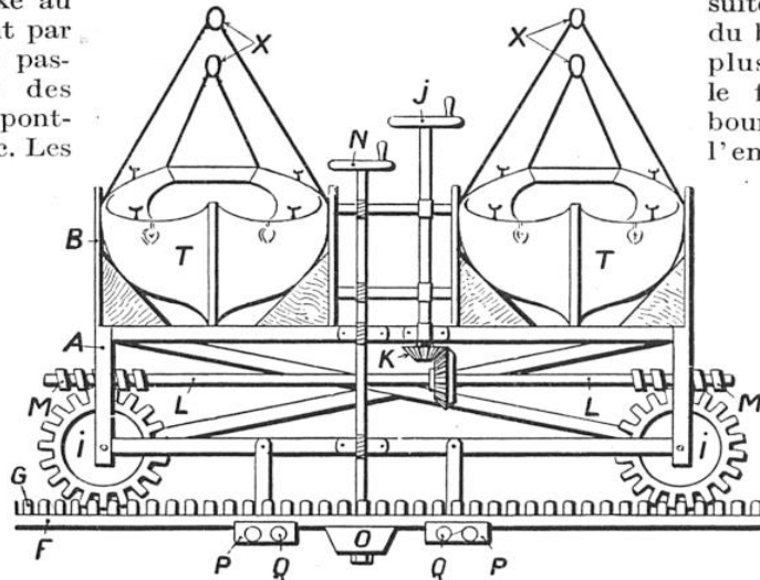
FIG. 3. — CHÂSSIS DE L'APPAREIL DE SAUVETAGE MARITIME DAULARD-BRION
