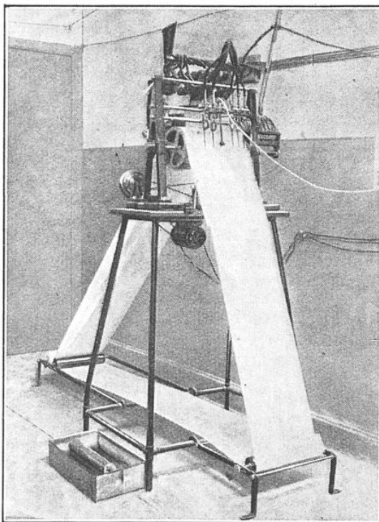
FIG. 2. — L'APPAREIL ENREGISTREUR EN ÉTAT DE MARCHÉ
