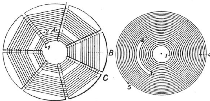
FIG. 4. — GALETS COMPORTANT LES TROIS ENROULEMENTS R. P. S. DE LA FIGURE 3
