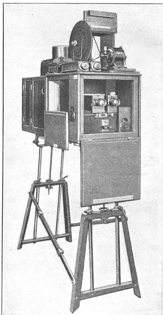
FIG. 4. — LE PULSOGRAPHE VU DE FACE
