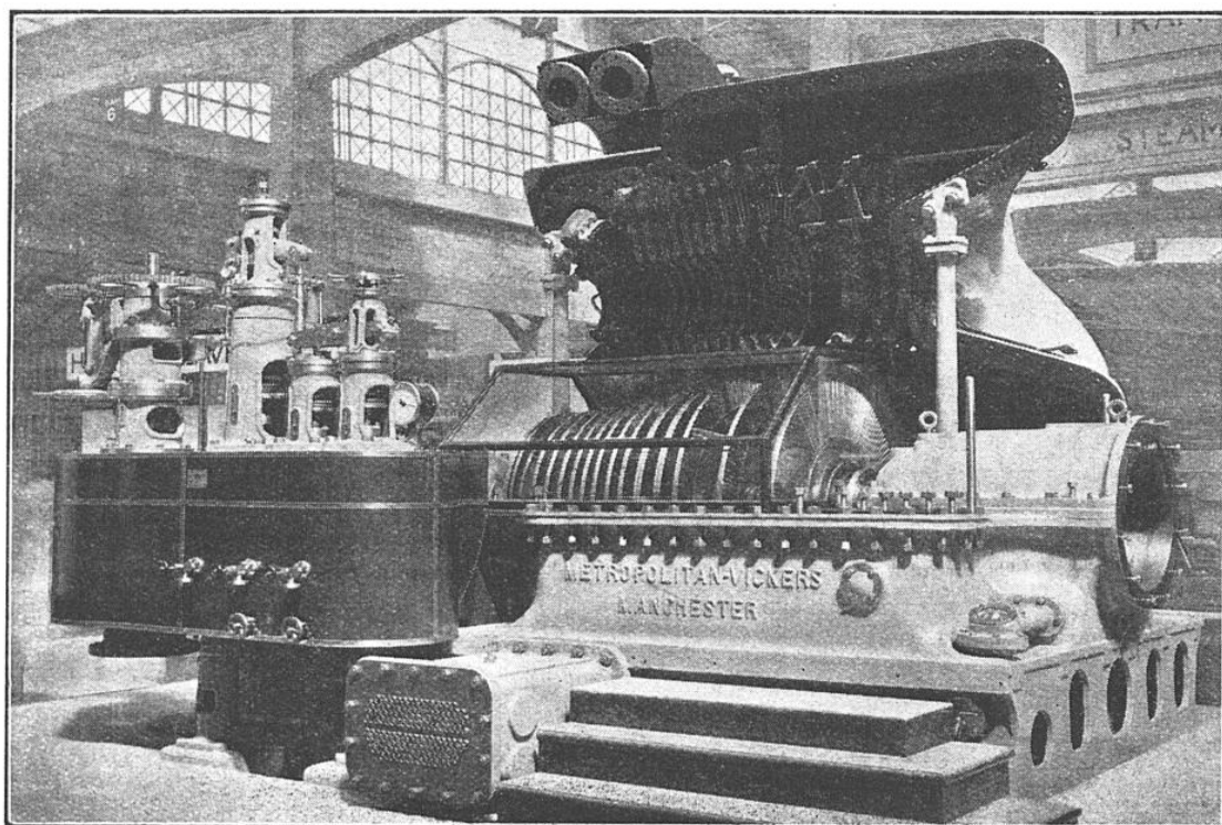
TURBINE A VAPEUR OUVERTE POUR EN MONTRER L'AGENCEMENT DU ROTOR ET DU STATOR
