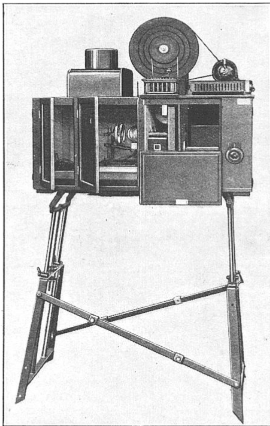
FIG. 5. — VUE LATÉRALE DU PULSOGRAPHE DAPONTE
