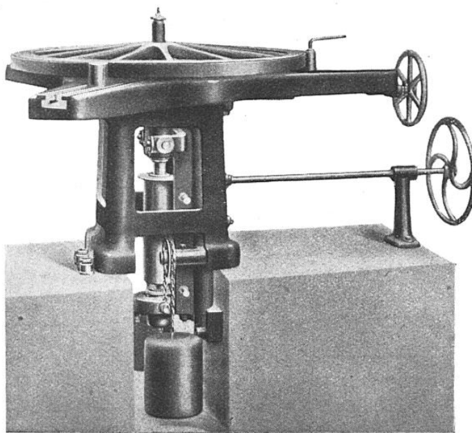
MACHINE A ALÉSER LES ROUES A MOYEURS MÉTALLIQUES
