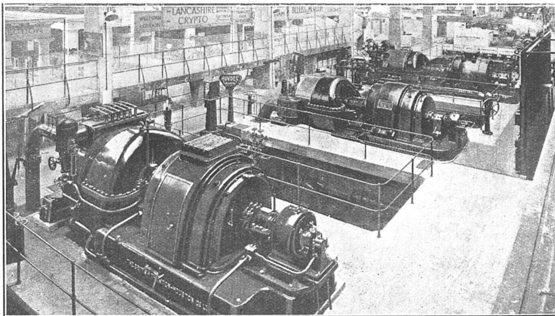
VUE DE LA CENTRALE ÉLECTRIQUE QUI ALIMENTE LA TOTALITÉ DE L'EXPOSITION
