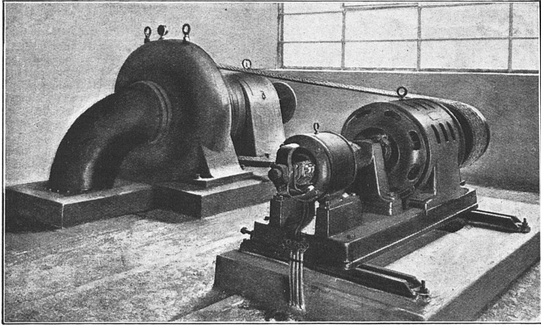
FIG. 3. — VUE D'UNE PETITE STATION HYDRO-ÉLECTRIQUE AUTOMATIQUE PRODUISANT DU COURANT A 3.000 VOLTS
