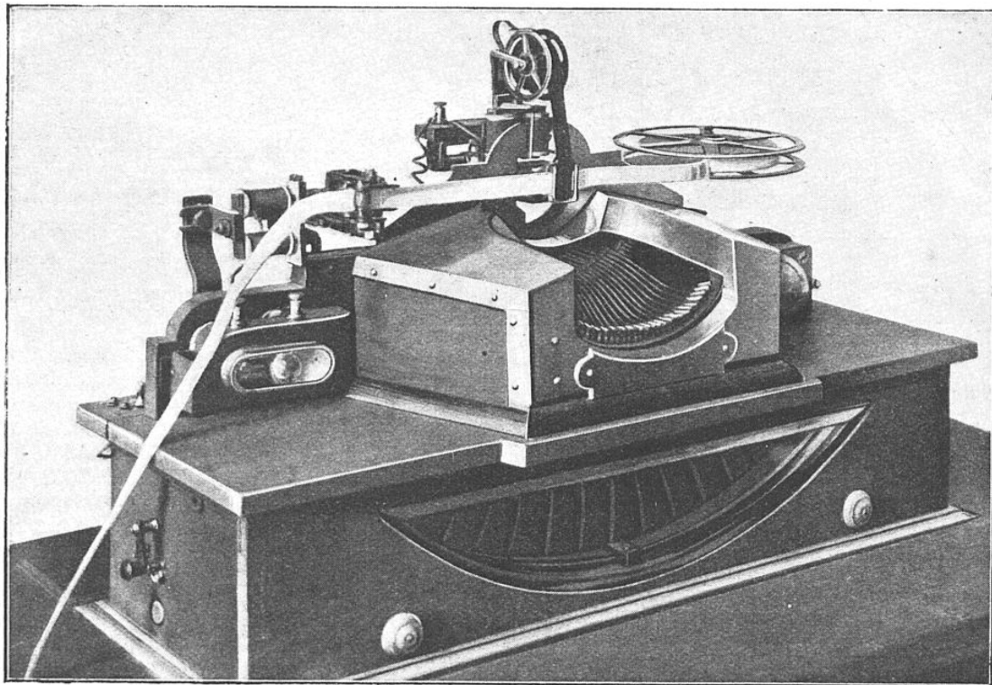
ORGANES RÉCEPTEURS DES MESSAGES TRANSMIS A DISTANCE
