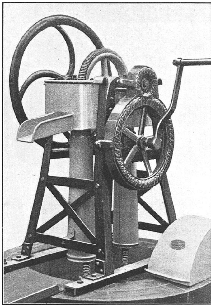
ÉLÉVATEUR D'EAU PAR CHAÎNE PLACÉ DIRECTEMENT SUR LA MARGELLE D'UN Puits
