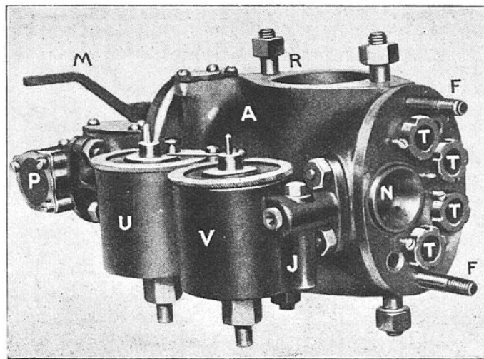
VUE D'ENSEMBLE DU CARBURATEUR OUVERT
