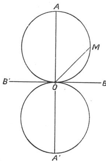
FIG. 2. — COURBE EN FORME DE 8 D'UN CADRE ÉMETTEUR
