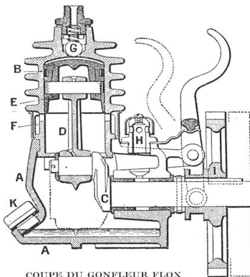
COUPE DU GONFLEUR FLOX
