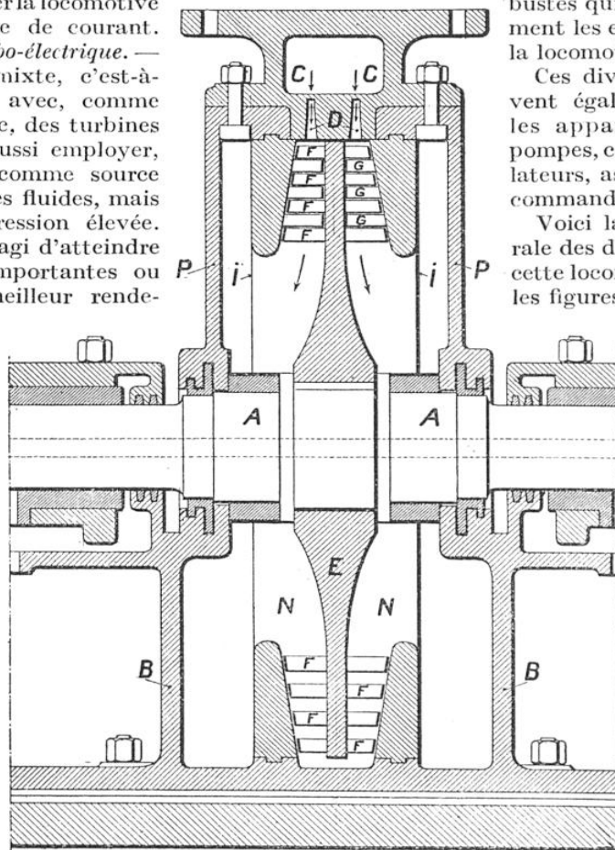
FIG. 3. — TURBINE CENTRIPÈTE A HAUTE PRESSION, SYSTÈME LÉON MÉTAIS
