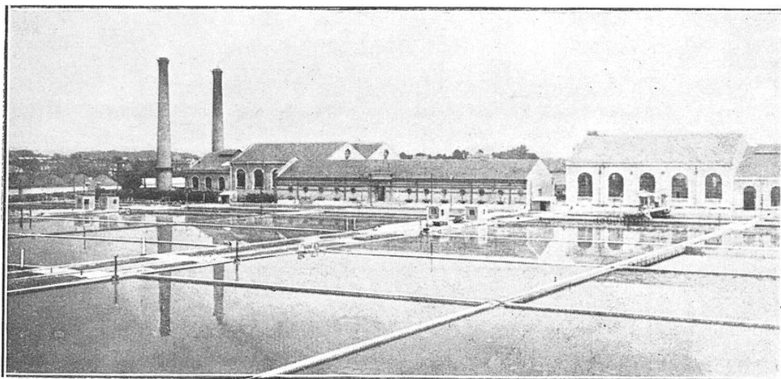
VUE D'ENSEMBLE DE L'USINE BASSE DE CHOISY-LE-ROI
