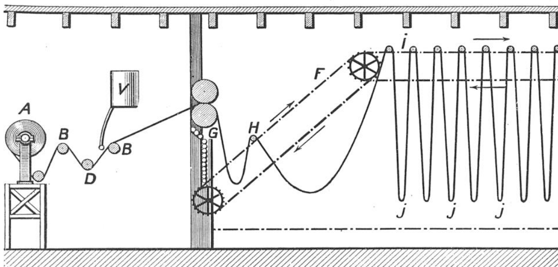
SCHÉMA DE LA PARTIE AVANT DE LA MACHINE LUMIÈRE POUR LA FABRICATION DU PAPIER AU GÉLATINO-BROMURE
