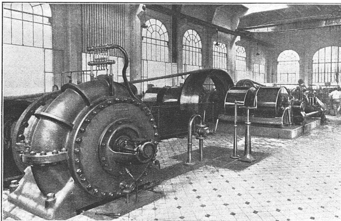
POMPE CENTRIFUGE COMMANDÉE PAR UN PUISSANT MOTEUR A GAZ PAUVRE
