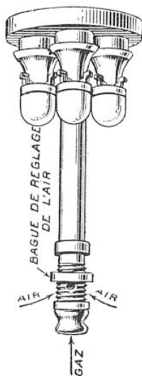
NOUVEAU BEC D'ÉCLAIRAGE A GRAND RENDEMENT ET FAIBLE CONSOMMATION
