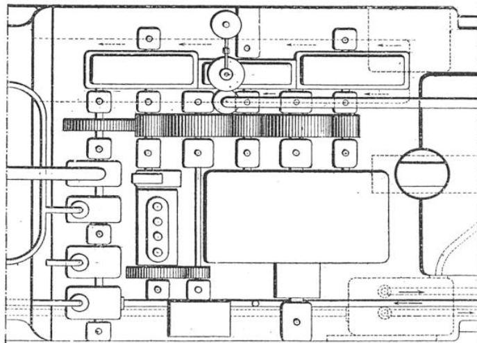
FIG. 6. — PLAN PARTIEL DE LA LOCOMOTIVE MIXTE DITE TURBO-ÉLECTRIQUE
