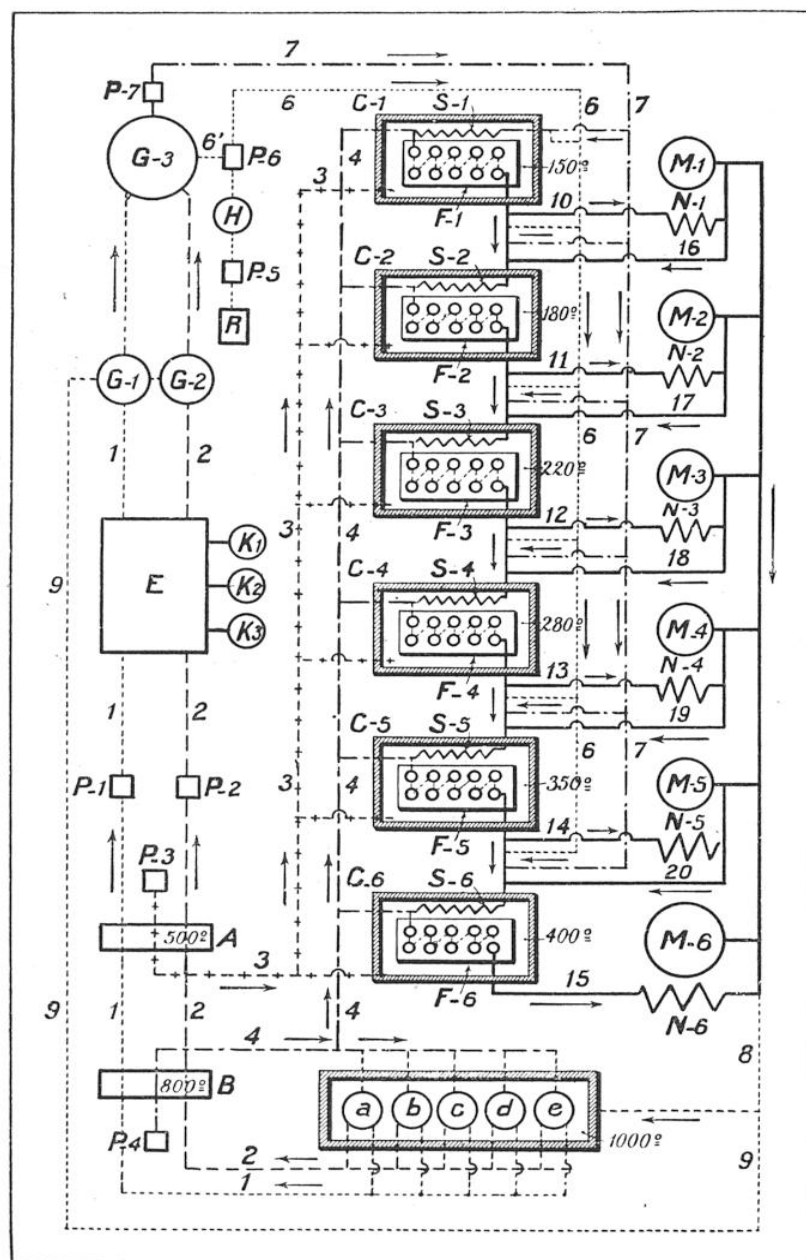
FIG. 6. — PLAN D'UNE USINE TYPE A FOURS CATALYSEURS POUR LA PRODUCTION DU PÉTROLE SYNTHÉTIQUE
