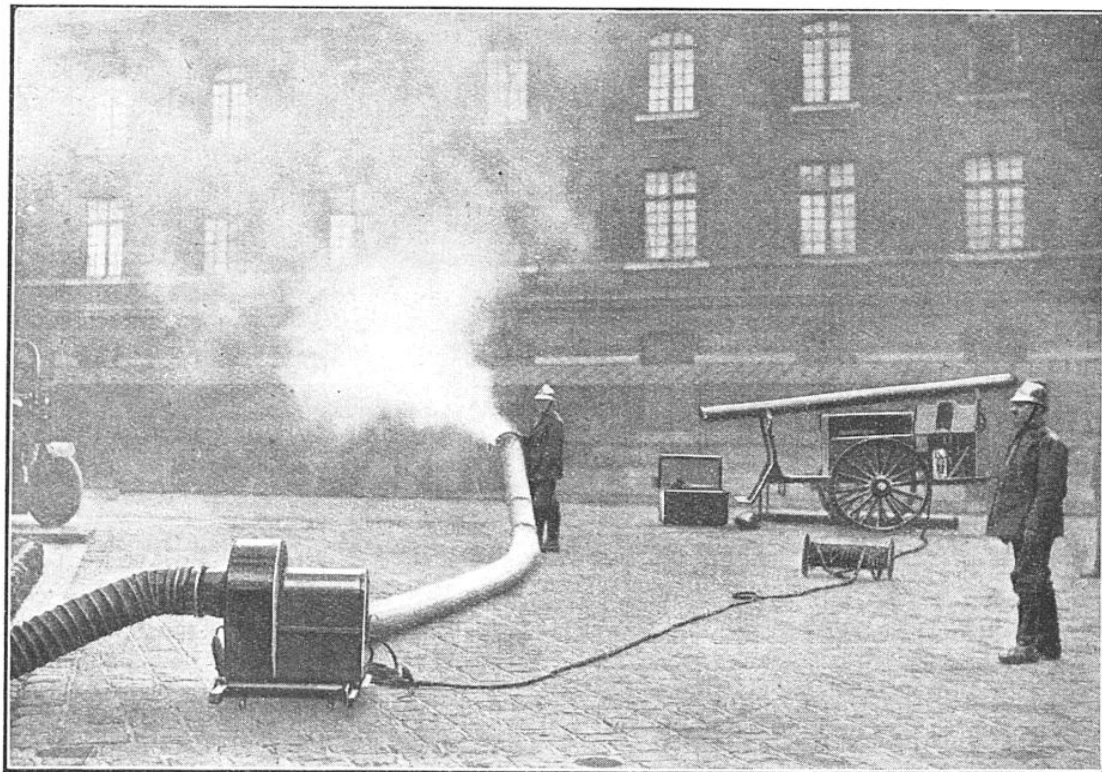
CETTE PHOTOGRAPHIE MONTRE LE VENTILATEUR EN PLEINE ACTION
