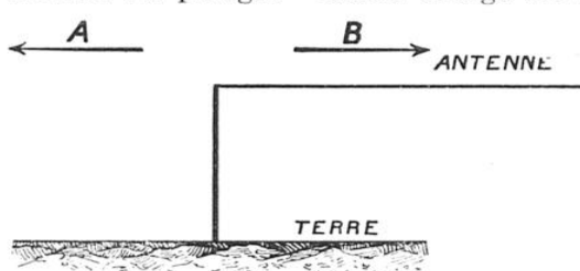
FIG. 1. — TYPE D'ANTENNE DIRIGÉE Avec une telle antenne, un correspondant situé dans la direction de la flèche de gauche recevra mieux les signaux qu'un correspondant situé dans la direction de la flèche B.
