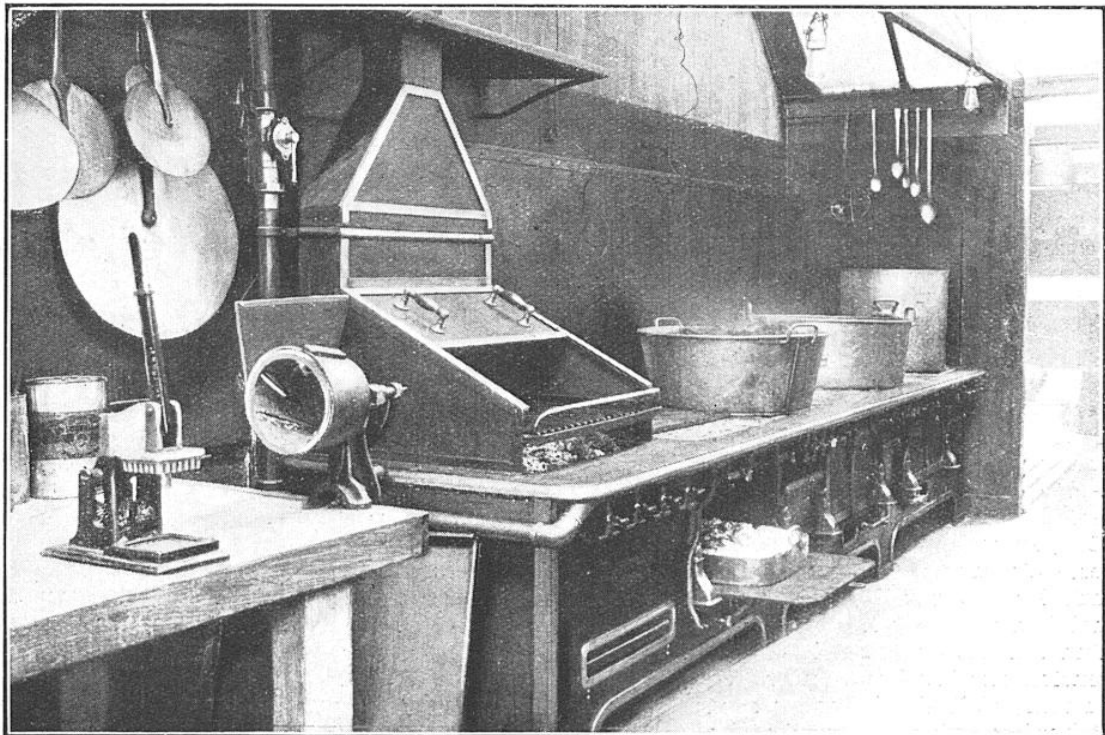
CUISINE DE RESTAURANT EXCLUSIVEMENT ALIMENTÉE AU GAZ
