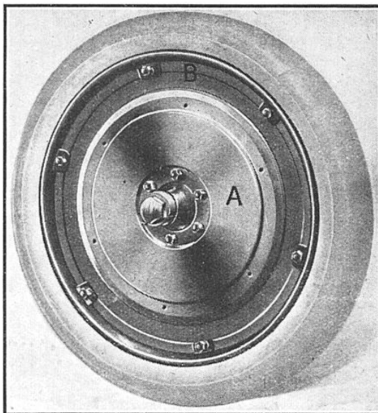
VUE EXTÉRIEURE DE LA ROUE COSTE A, plaque extérieure en acier, solidaire du moyeu ; B, disque central en fibre, supportant la jante.
