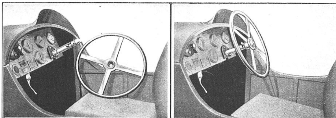
DEUX POSITIONS DU VOLANT AMOVIBLE IMAGINÉ PAR M. LAPAIRE A droite, le volant dans sa position normale ; à gauche, le volant retiré. Sur le tube de direction, on distingue la broche à baïonnette qui sert au verrouillage de l'appareil.
