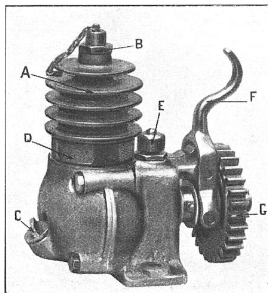
VUE EXTÉRIEURE DU GONFLEUR FLOX
