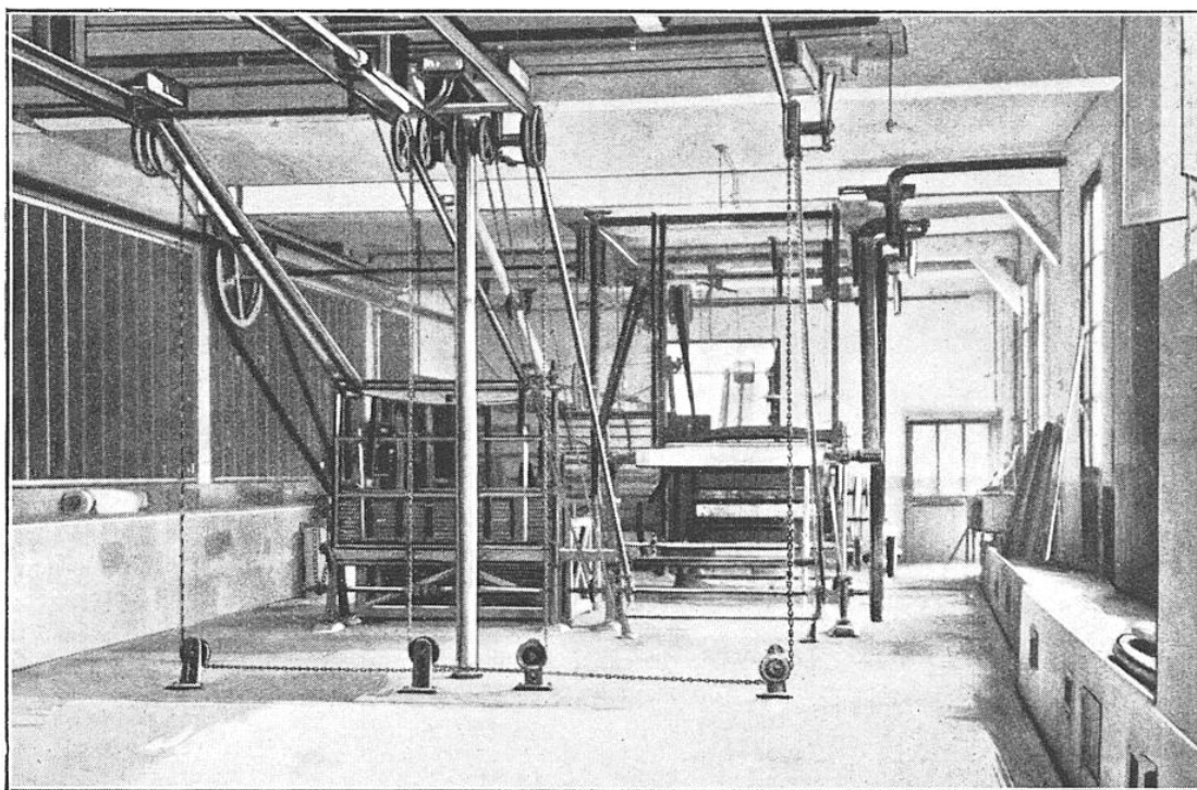
MACHINE POUR LA FABRICATION DU PAPIER AU GÉLATINO-BROMURE (PHOTOGRAPHIE PRISE DANS LES ÉTABLISSEMENTS MICHEL ET PAILLOT)
