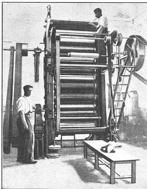
CALANDRE POUR DONNER AU PAPIER BARYTÉ UN BON GLAÇAGE AVANT D'Y APPLIQUER L'ÉMULSION
