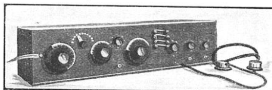
LE DÉTECTEUR-AMPLIFICATEUR (A DROITE) MIS A LA SUITE D'UN APPAREIL CONTENANT UN CIRCUIT D'ACCORD ET DEUX LAMPES HAUTE FRÉQUENCE
