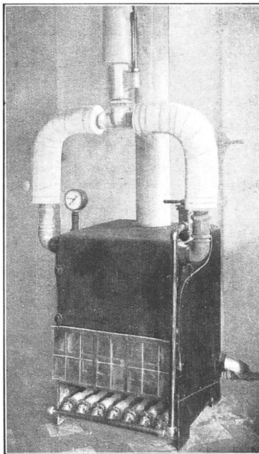
CHAUDIÈRE A GAZ POUR LE CHAUFFAGE CENTRAL A L'EAU CHAUDE OU A LA VAPEUR BASSE PRESSION ET POUR LA DISTRIBUTION DE L'EAU CHAUDE, SYSTÈME « PHI »
