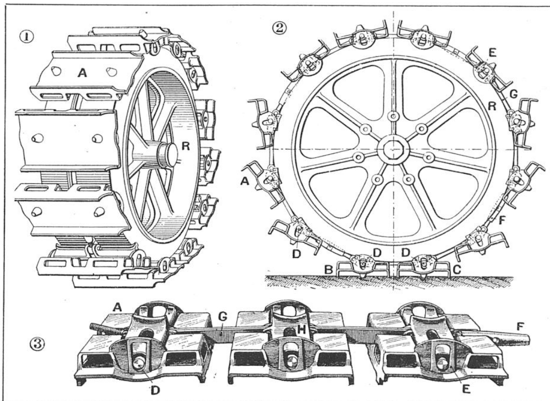
SABOTS ARTICULÉS, AMOVIBLES, POUR DONNER L'ADHÉRENCE AUX ROUES MOTRICES
