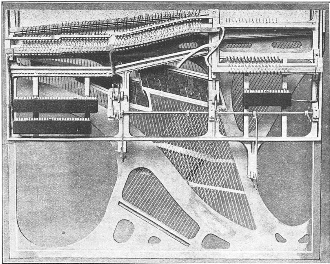
FIG. 2. — VUE INTÉRIEURE, ARRIÈRE, DU PIANO ÉQUIPÉ ÉLECTRIQUEMENT
