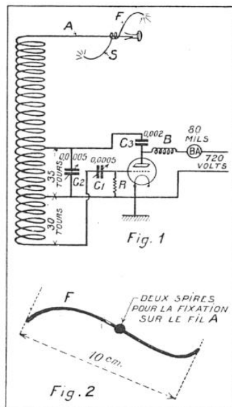
PLANCHE 2. — SCHÉMAS DE CONSTRUCTION DU MODULATEUR REINARTZ
