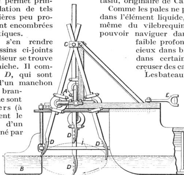
FIG. 1. — DISPOSITION DU PROPULSEUR ANASTASIU A L'ARRIÈRE D'UNE PÉNICHE
