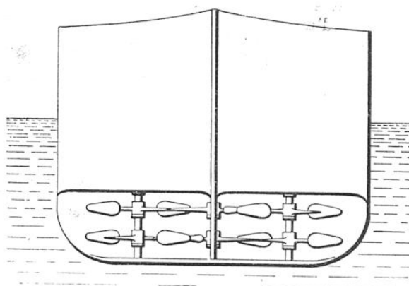
FIG. 5. — DISPOSITION, VUE EN BOUT, DES PALES ROTATIVES, SYSTÈME JOURDAIN
