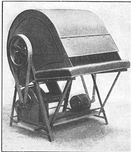
EN MÊME TEMPS QU'ELLE BAT, CETTE MACHINE ASPIRE LES POUSSIÈRES, POILS DÉTACHÉS, RÉSIDUS, ETC., ET LES REFOULE À L'EXTÉRIEUR DANS UN SAC
