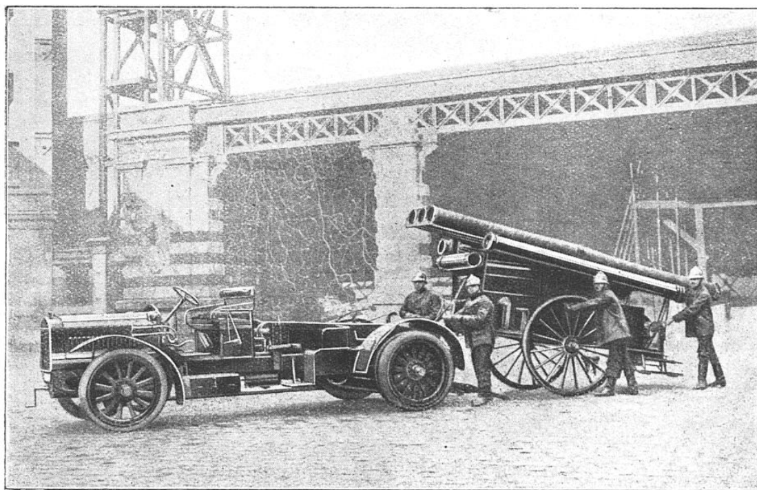
LE GROUPE VENTILATEUR EST MONTÉ SUR UN CHARIOT PORTEUR D'ÉCHELLE DANS LES MÊMES CONDITIONS QUE CELLE-CI
