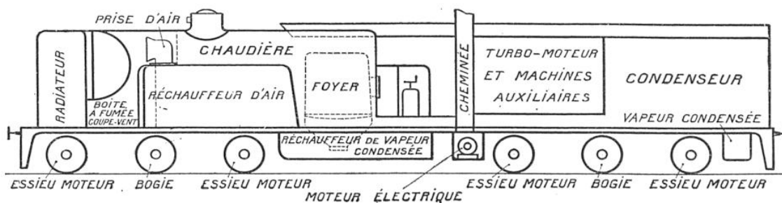
FIG. 1 — ENSEMBLE DE LA TURBO-LOCOMOTIVE ÉLECTRIQUE MÉTAIS
