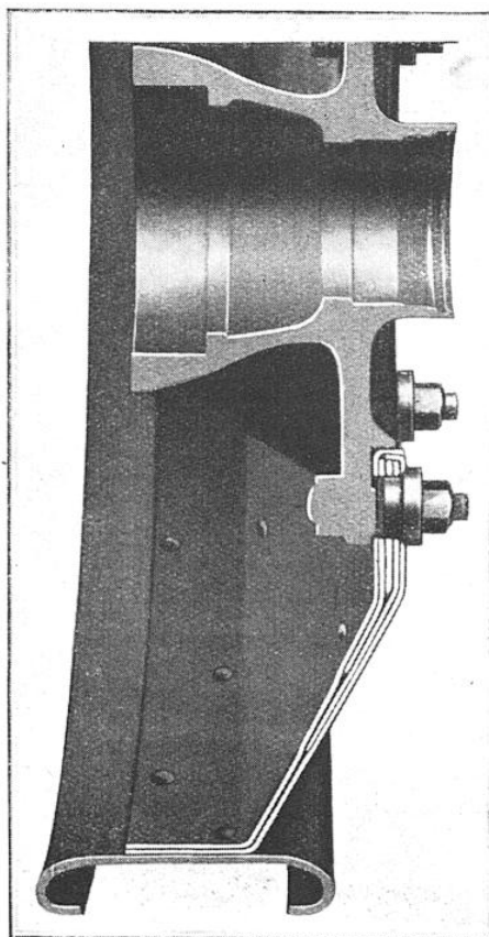
COUPE DE LA ROUE PLEINE « O. D. »
