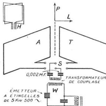
FIG. 4. — SCHÉMA DE L'ENSEMBLE DES RADIOPHARES DIRECTIFS
