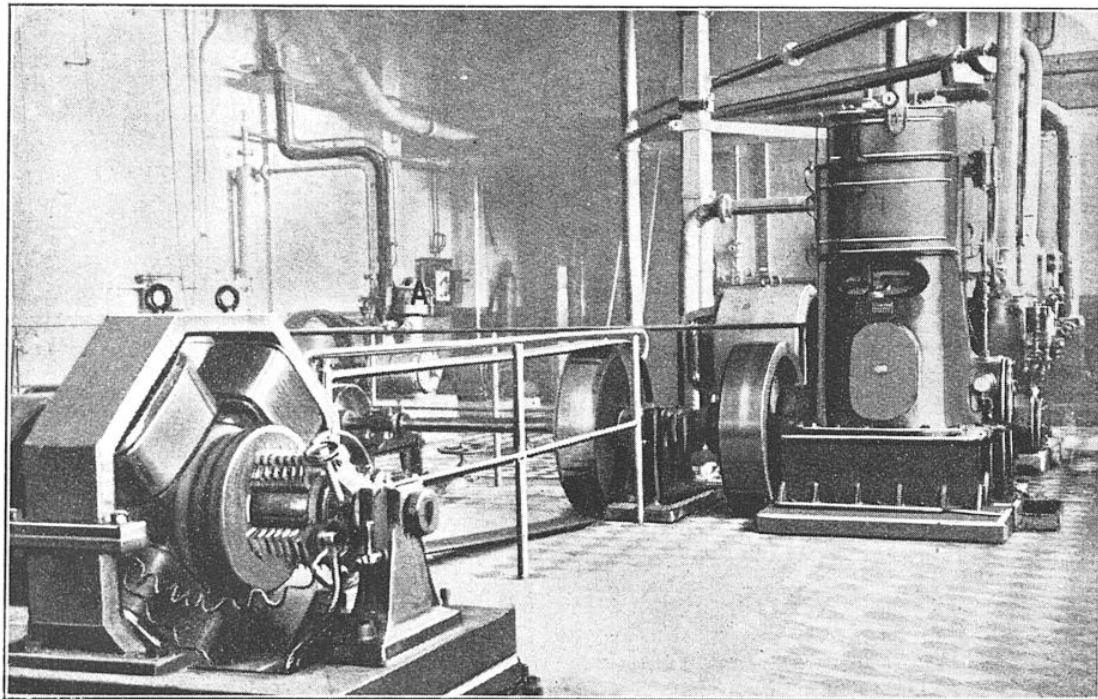
SALLE DES MACHINES D'UNE FABRIQUE DE PAPIERS PHOTOGRAPHIQUES
