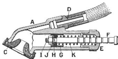
RACCORD INDICATEUR DE PRESSION DU GONFLEUR FLOX
