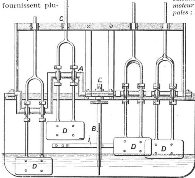
FIG. 2. — DÉTAIL DU PROPULSEUR ANASTASIU
