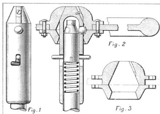
DÉTAILS DE CONSTRUCTION ET DE FONCTIONNEMENT DU VOLANT AMOVIBLE J. LAPAIRE (On trouvera dans le texte, à la page suivante, la description des figures.)
