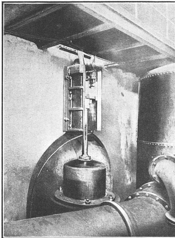
LA POMPE NOURRICIÈRE
