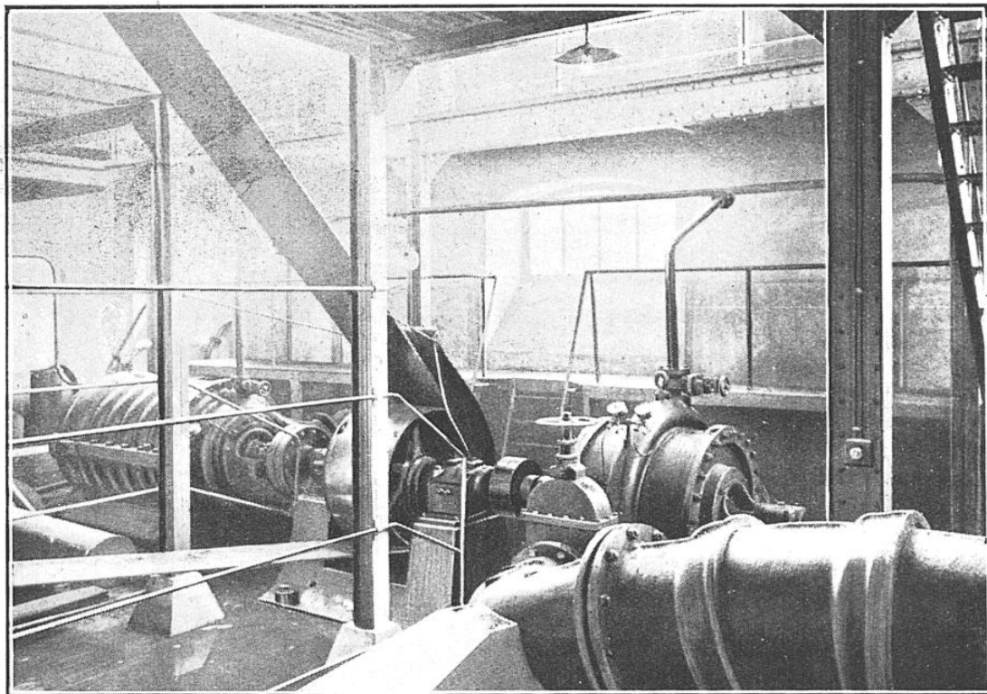
LES POMPES CENTRIFUGES RATEAU, COMMANDÉES PAR L'UNE DES MACHINES A GRANDE VITESSE QU'ON VOIT SUR LA PHOTOGRAPHIE PAGE 276
