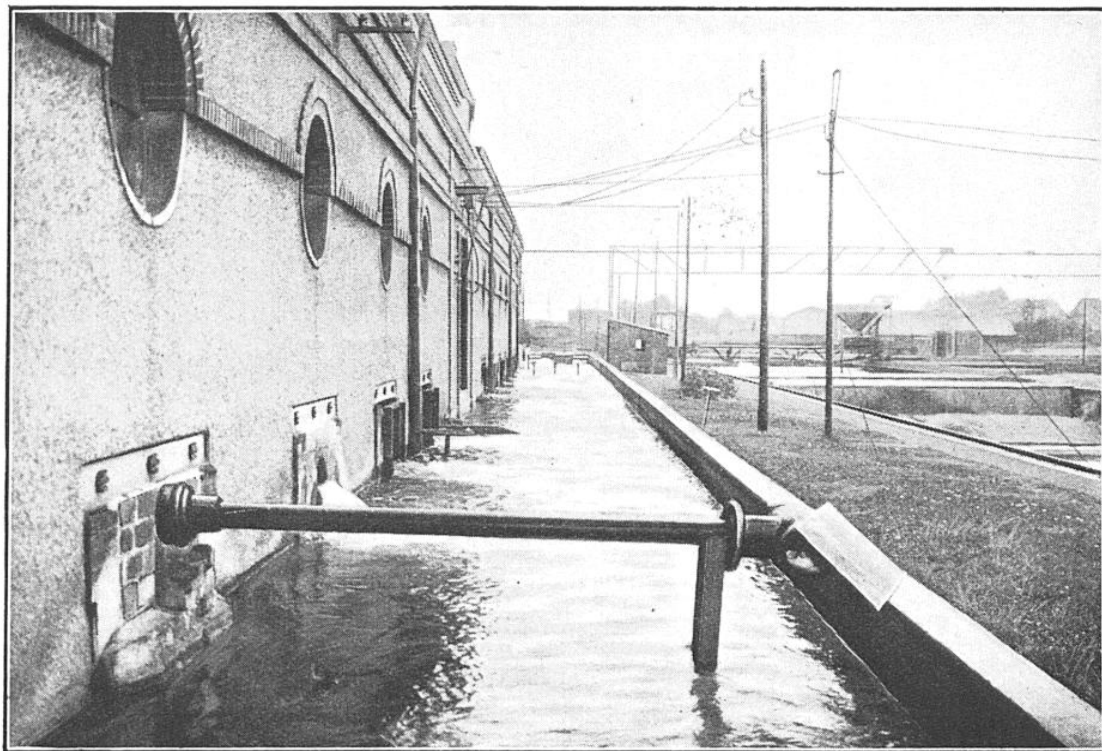
VUE PERSPECTIVE D'UNE COULOTTE D'AMENÉE DE L'EAU DE SEINE C'est par cette sorte de canal que passe l'eau, encore brute, lorsqu'elle se trouve refoulée par les pompes nourricières aux bassins préfiltrants et filtrants.
