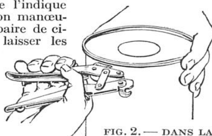
FIG. 2. — DANS LA FENTE ON ENGAGE LA LAME DE LA CISAILLE, PUIS ON DÉCOUPE RÉGULIÈREMENT SOUS LE COUVERCLE
