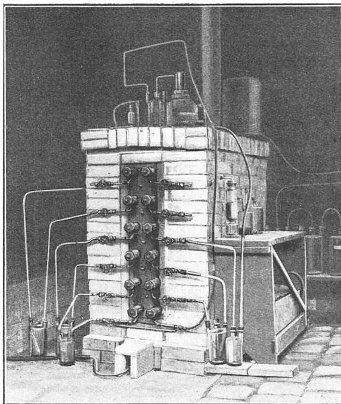
FIG. 3. — LE FOUR DE CATALYSE POUR L'OBTENTION DU PÉTROLE SYNTHÉTIQUE
