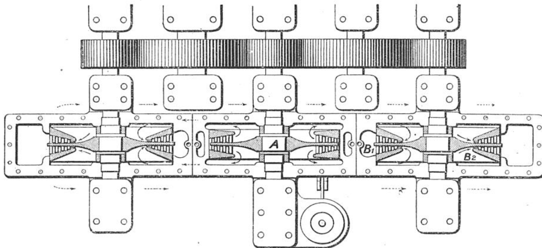
FIG. 2. — COUPE SUIVANT L'AXE DES TURBINES DE LA LOCOMOTIVE MÉTAIS
