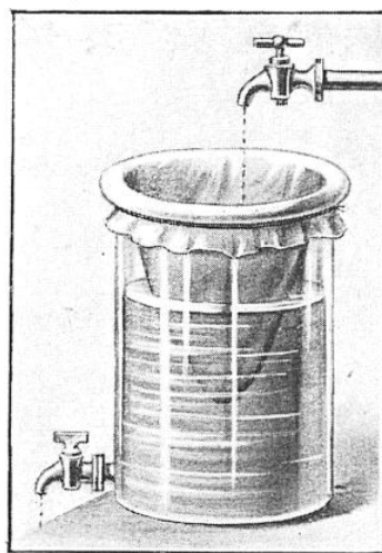
LAVAGE DE L'ÉMULSION DANS UNE CHAUSSE EN FEUTRE
