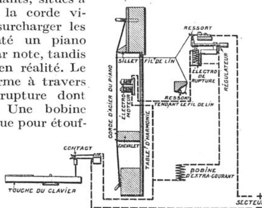
FIG. 3. - SCHÉMA DU MONTAGE ÉLECTRIQUE
