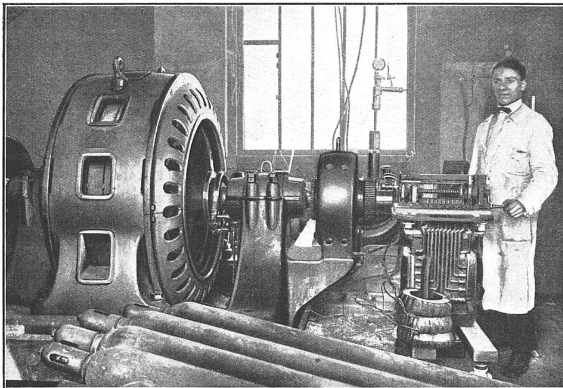
FIG. 7. — ALTERNATEUR DE 80 KILOWATTS FOURNISSANT LE COURANT ALTERNATIF A HAUTE TENSION POUR LA PRODUCTION DU PÉTROLE SYNTHÉTIQUE
