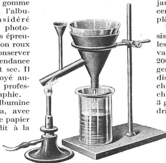
ENTONNOIR A FILTRATION CHAUDE
