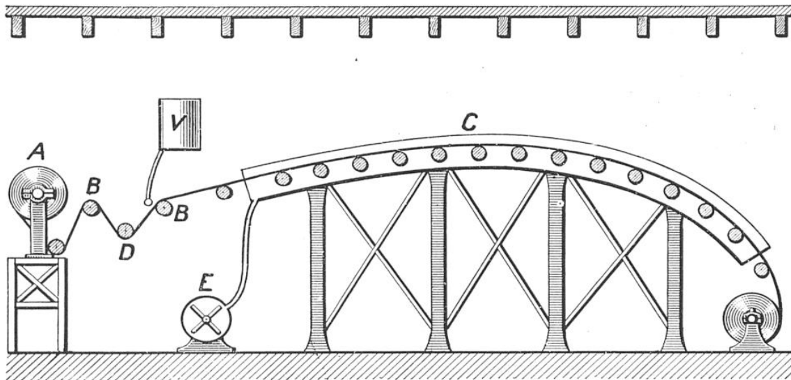
SCHÉMA DE LA MACHINE POUR FABRIQUER LE PAPIER AU CITRATE
