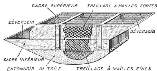
LE TRIEUR DE POMMES DE TERRE, A SECOUSSES, DE M. NIQUET-HÉSÈQUE
