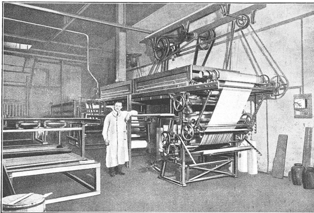
MACHINE HAUSSAIRE POUR LA PRÉPARATION INDUSTRIELLE DU PAPIER AU FERRO-PRUSSATE, DIT « BLEU », ET AU FERRO-GALLATE
