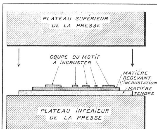
FIG. 1. — ILLUSTRATION SCHEMATIQUE DU PROCÉDÉ D'INCRUSTATION MAX WOLFERS
