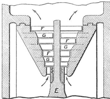
FIG. 5. — DISTRIBUTION DES AUBAGES DE LA TURBINE CENTRIFUGE Cette figure montre une variante comprenant des aubes spéciales pouvant être montées sur la couronne mobile E (voir fig. 2) ; F, aubes mobiles (rotor) ; G, aubes directrices (stator) de la turbine centrifuge (BP) de la turbo-locomotive. La vapeur BP pénètre près de l'axe par des tuyères d'admission et son travail a lieu suivant le sens des flèches.
