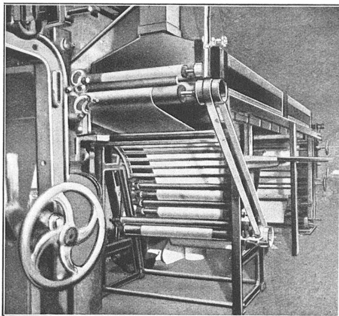
VUE ARRIÈRE DE LA MACHINE PRÉCÉDENTE MONTRANT LE PASSAGE DU PAPIER ENTRE LES ROULEAUX
