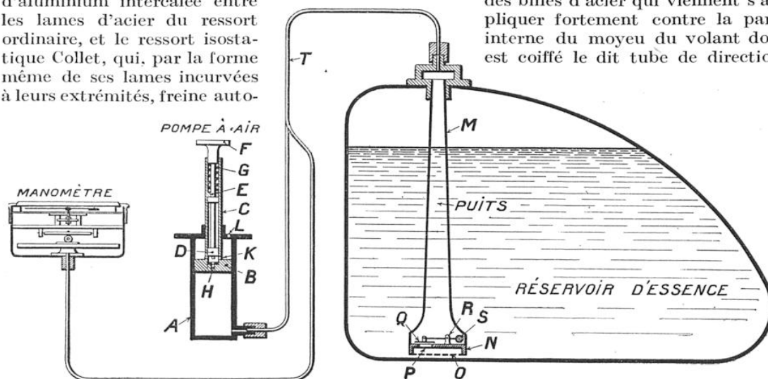
SCHEMA GÉNÉRAL DE MONTAGE DE LA JAUGE D'ESSENCE « O. S. »
