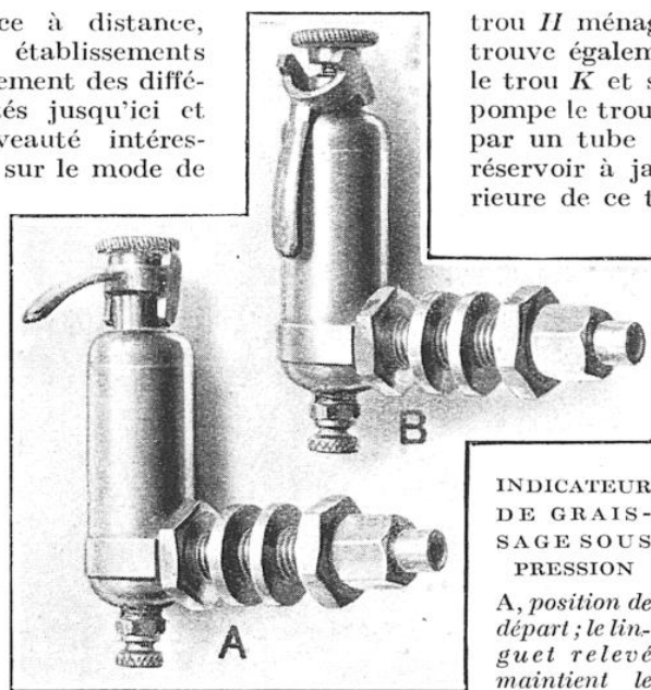
pareil ; B, position d'arrêt ; le graissage étant interrompu, le piston, n'étant plus soutenu par la pression de l'huile, est retombé, coupant le circuit.
