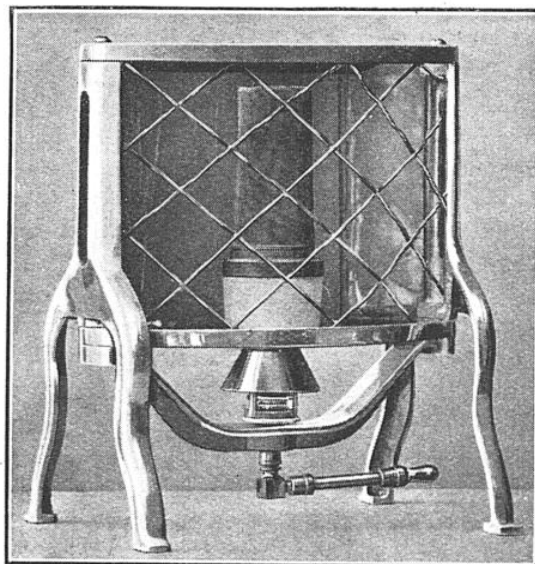
RADIATEUR ET RÉCHAUD COMBINÉS, A MANCHON DROIT EN TOILE MÉTALLIQUE
