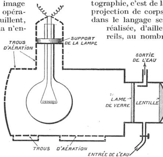
FIG. 3. — COUPE DU PROJECTEUR THUILLANT
