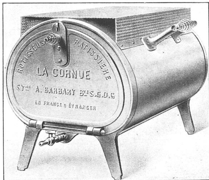
FOUR A GAZ INDÉPENDANT POURVU D'UN GRIL ET SURMONTÉ D'UN CHAUFFE-PLATS OU ASSIETTES
