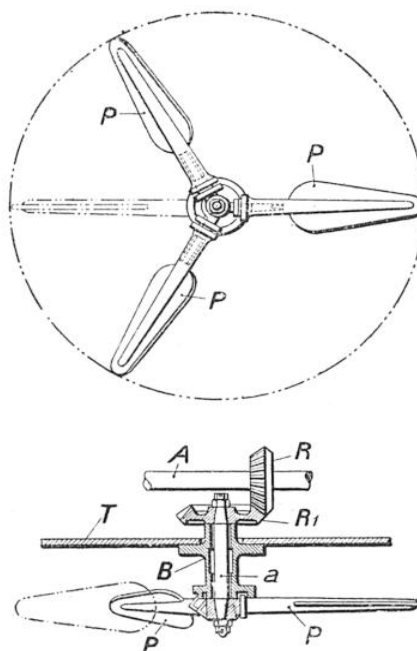
FIG. 3. — PROPULSEUR A RAMES OU A PALES ROTATIVES, SYSTÈME JOURDAIN
