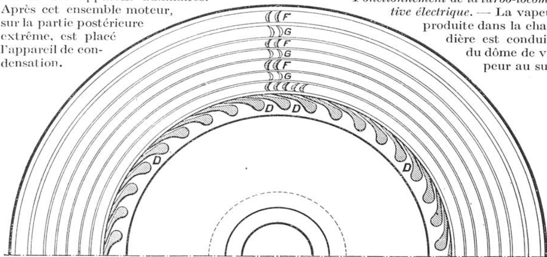
FIG. 4. — CARTER SUPÉRIEUR DE LA TURBINE CENTRIFUGE A BASSE PRESSION F, aubes mobiles formant rotor ; G, aubes directrices (stator) de la turbine centrifuge (BP), système Léon Métals ; D, tuyères d'admission de la vapeur à basse pression.
