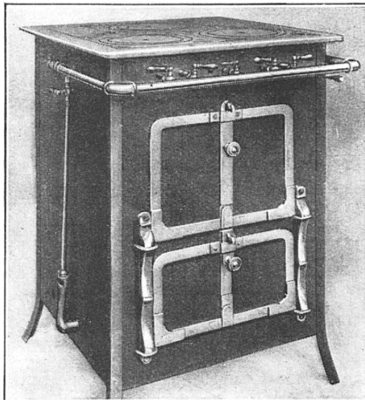
CUISINIÈRE A GAZ POURVUE D'UN FOUR, D'UN SECOND FOUR-ROTISSOIRE ET D'UN DESSUS UNIFORMANT TABLE CHAUFFANTE, SYSTÈME « PHI »
