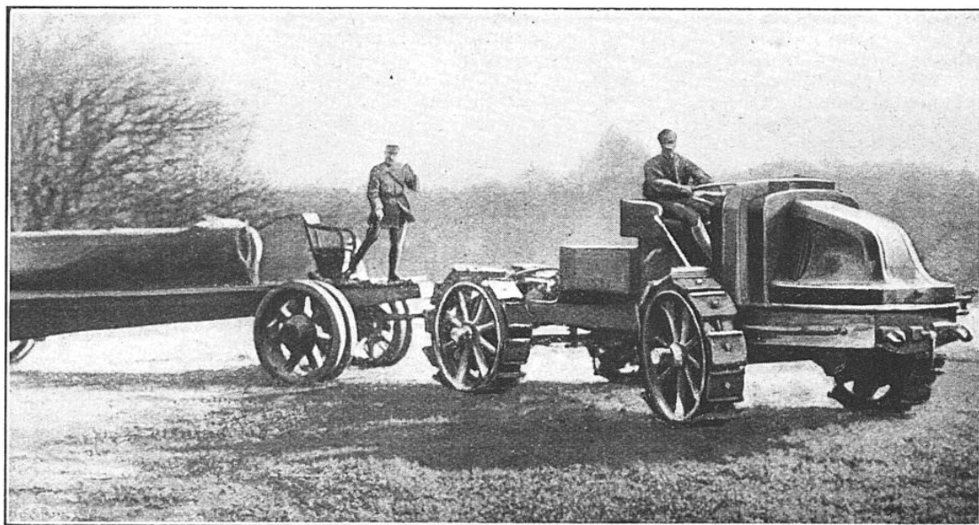
TRACTEUR MILITAIRE DONT LES ROUES SONT MUNIES DE SABOTS D'ADHÉRENCE GUERRINI
