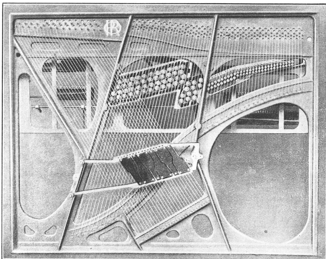
FIG. 4. — VUE INTÉRIEURE, AVANT, LA TABLE D'HARMONIE ENLEVÉE
