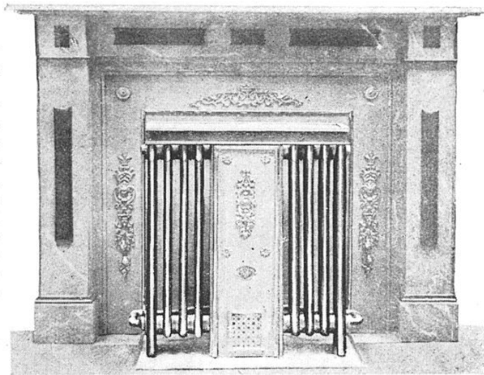
TYPE DE RADIATEUR A EAU CHAUDE ALIMENTÉ PAR LE GAZ D'ÉCLAIRAGE, SYSTÈME « AUTO-CALORIE »
