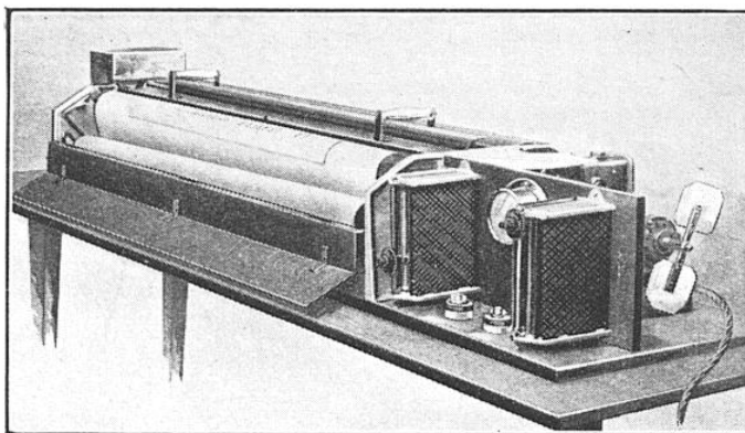
VUE EXTÉRIEURE DE L'ÉLECTROGRAPHE REX
