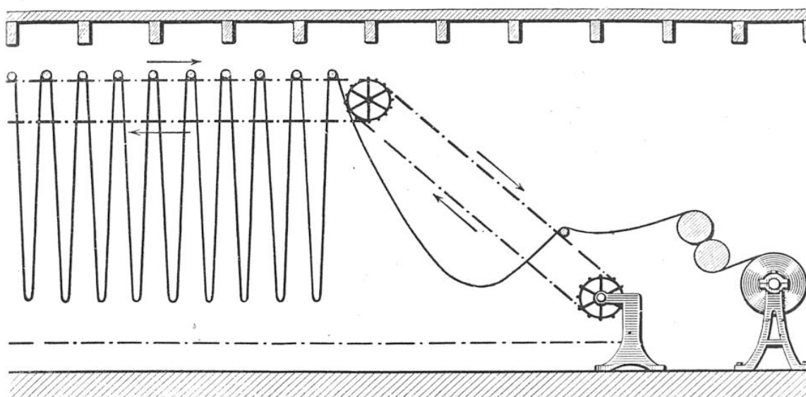
PARTIE ARRIÈRE DE LA MACHINE LUMIÈRE, MONTRANT L'ENROULEMENT DU PAPIER ÉMULSIONNÉ ET SÉCHÉ APRÈS SON PASSAGE ENTRE DEUX ROULEAUX FEUTRÉS ENTRAÎNEURS
