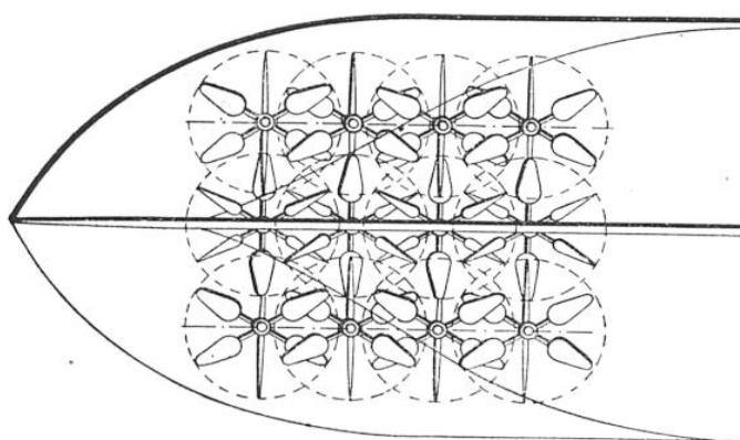
FIG. 6. — VUE EN DESSOUS DE L'INSTALLATION DES PALES JOURDAIN TOURNANT DANS UN CERCLE
