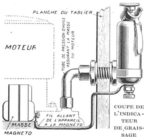
Dans cette figure, le linguet étant abaissé indique le bon fonctionnement du graissage pendant la marche du moteur.
