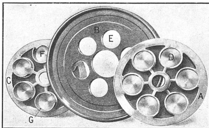
PIÈCES CONSTITUANT LA NOUVELLE ROUE A et C, flasques extérieurs retournés montrant les alvéoles où sont logés les ressorts G ; B, disque central percé de trous pour le passage des ressorts et du moyeu ; D, F, alvéoles des ressorts ; E, passage des ressorts dans le disque central.
