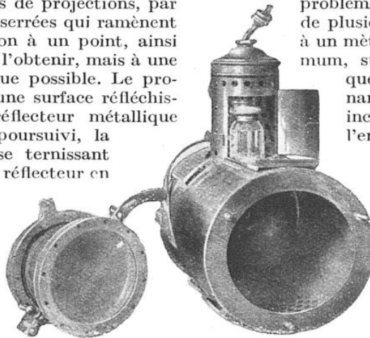
FIG. 4. — LE PROJECTEUR DÉMONTÉ A droite, le logement de la lampe surmonté de la lanterne ouverte ; à gauche, la chambre de circulation d'eau qui se fixe à l'avant de la première partie.
