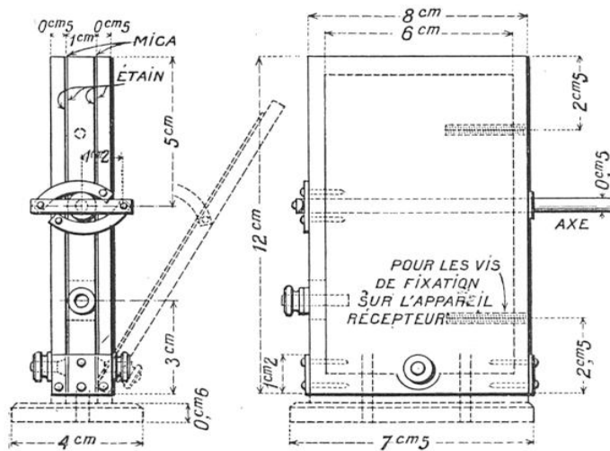
SCHEMA DE CONSTRUCTION D'UN CONDENSATEUR VARIABLE
