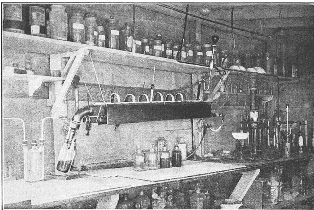
FIG. 5. — VUE INTÉRIEURE DU LABORATOIRE PROVISOIRE D'HYDROGÉNATION
