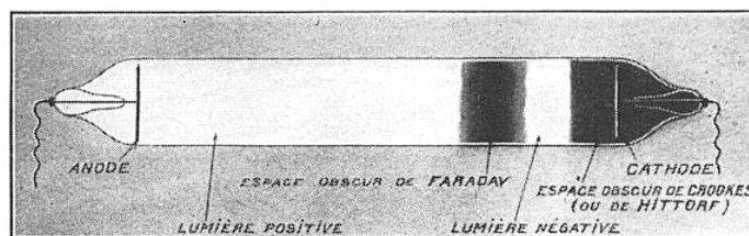
FIG. 2. — CURIEUSE RÉPARTITION DE LA LUMIÈRE DANS UN TUBE A DEUX ÉLECTRODES RENFERMANT UN GAZ SOUS UNE FAIBLE PRESSION
