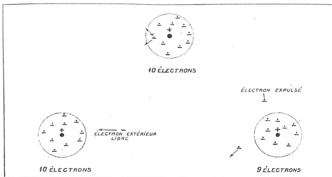
FIG. 1. — ILLUSTRATION SCHÉMATIQUE DU PHÉNOMÈNE DE L'IONISATION
