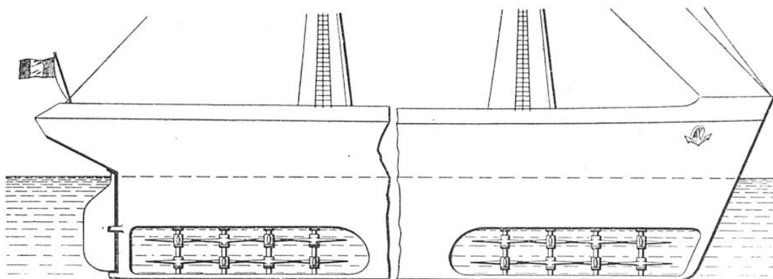
FIG. 4. — VUE AVANT ET VUE ARRIÈRE DU PROPULSEUR A PALES ROTATIVES
