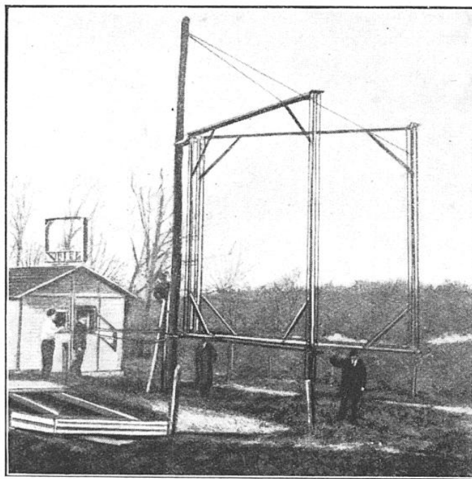
FIG. 3. — ENSEMBLE DE RADIOPHARES MOBILES AUTOUR D'UN AXE VERTICAL
