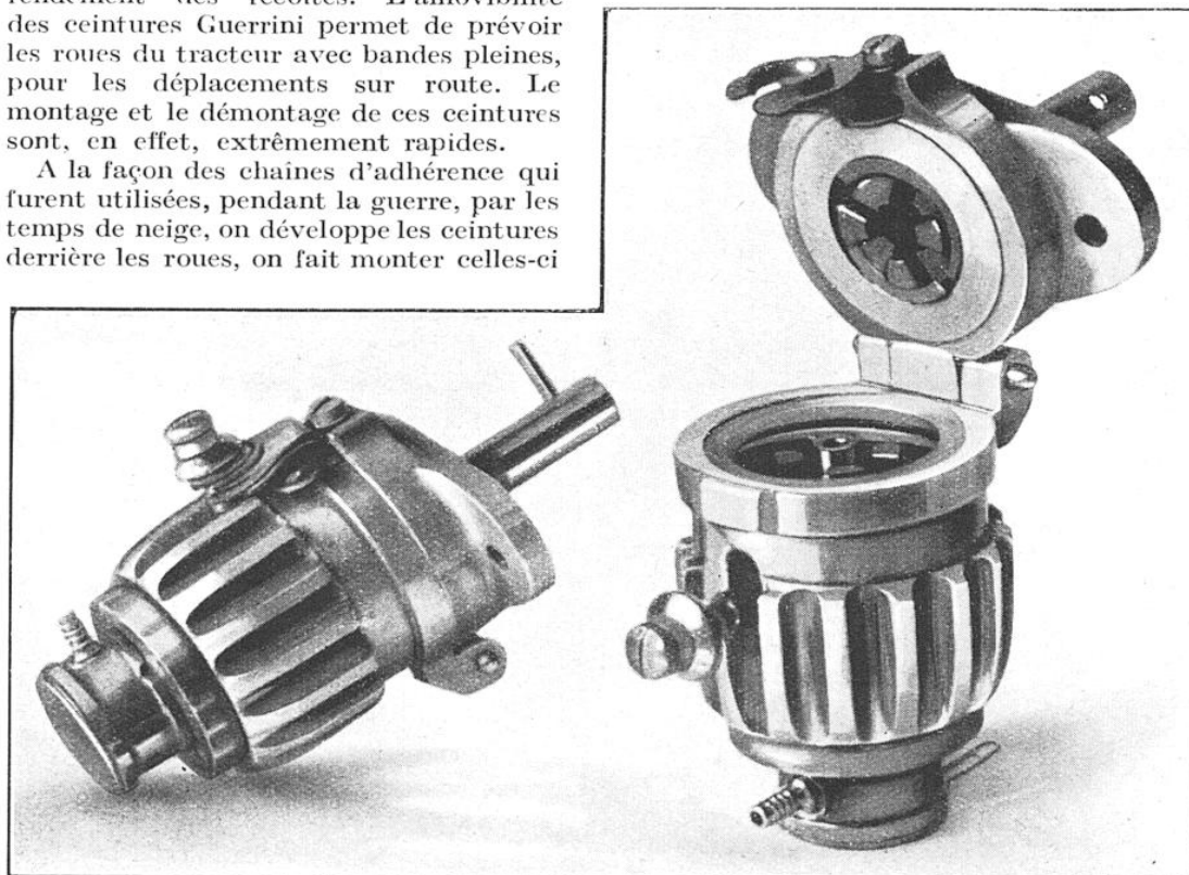
VUE EXTÉRIEURE DU GONFLEUR DE PNEUMATIQUES SAUSSARD
