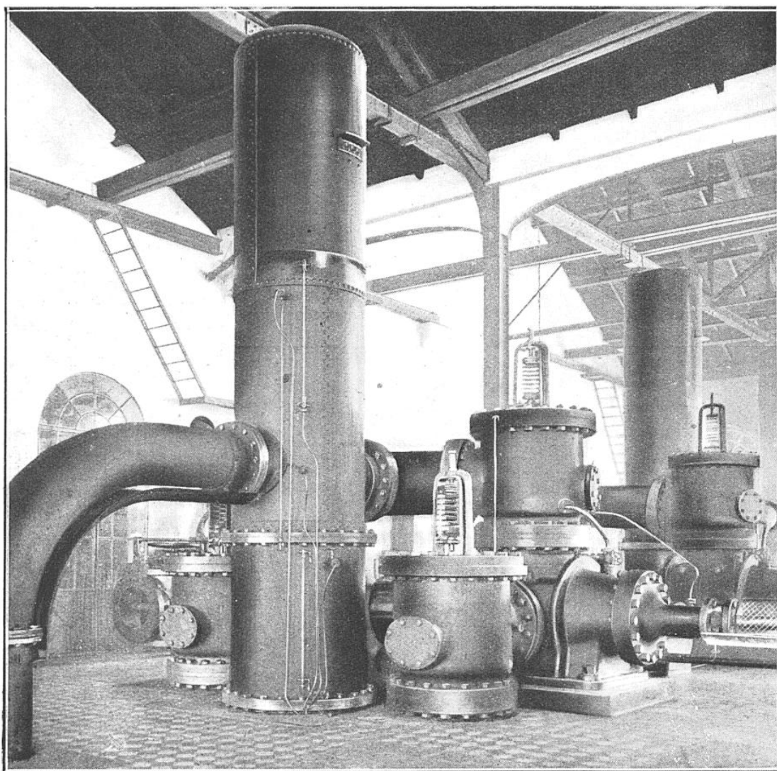
POMPE ÉLÉVATOIRE SYSTÈME FARCOT, COMMANDÉE DIRECTEMENT PAR L'UNE DES MACHINES QU'ON VOIT SUR LA PRÉCÉDENTE PHOTOGRAPHIE
