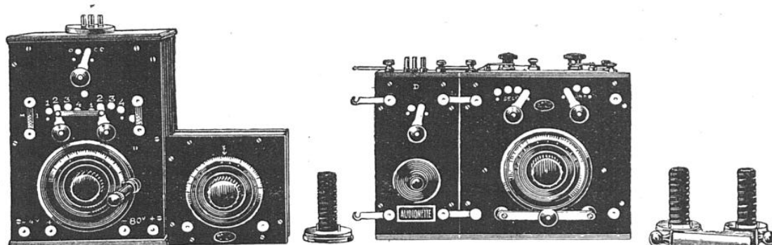
ÉLÉMENTS "SUPERHÉTÉRODYNETTE"
