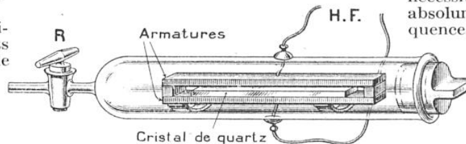
FIG. 5. — DISPOSITIF DES DOCTEURS GIEBE ET SCHEIBE, PERMETTANT L'OBSERVATION DIRECTE DES OSCILLATIONS DU QUARTZ
