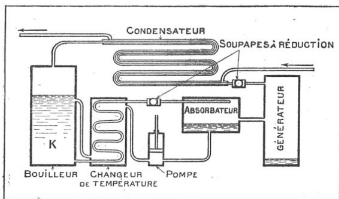
FIG. 3. — SCHÉMA DE FONCTIONNEMENT DE LA MACHINE FRIGORIFIQUE À ABSORPTION « CARRÉ »
