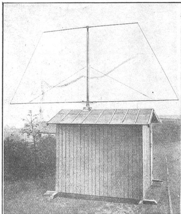
INSTALLATION D'ENSEMBLE D'UN POSTE DE RADIOGONOMÉTRIE
