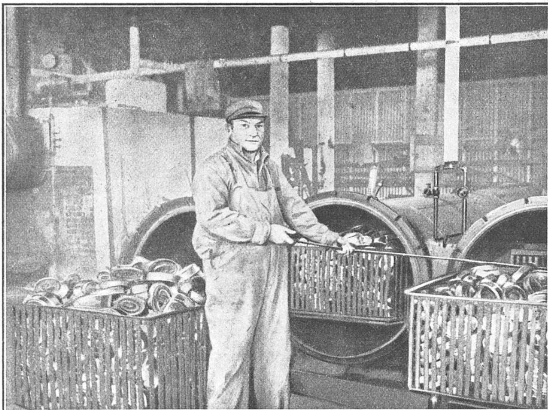
FIG. 8. — LES BOÎTES SERTIES SONT STÉRILISÉES PAR UN SÉJOUR DE DEUX HEURES DANS UN AUTOCLAVE CHAUFFÉ A 115 DEGRÉS
