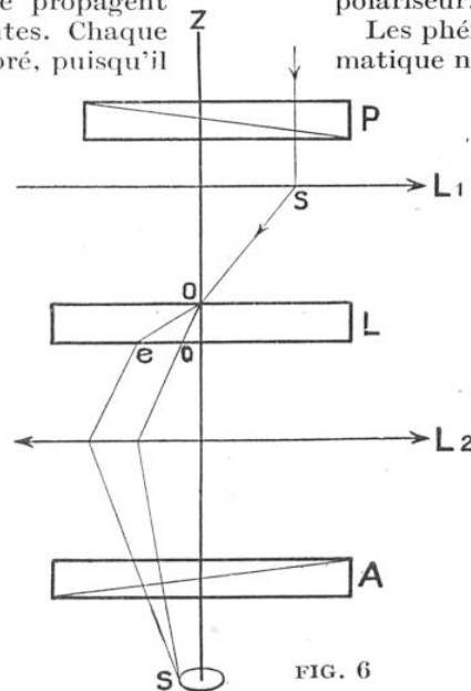
FIG. 6 SCHÉMA DU MICROSCOPE POLARISANT P, polariseur ; L_1 , lentille ; L, lame de cristal ; L_2 , lentille ; A, analyseur. Le rayon lumineux SO se divise en deux, Oe Oo , qui, à travers L_2 et A, donnent l'image colorée S.
