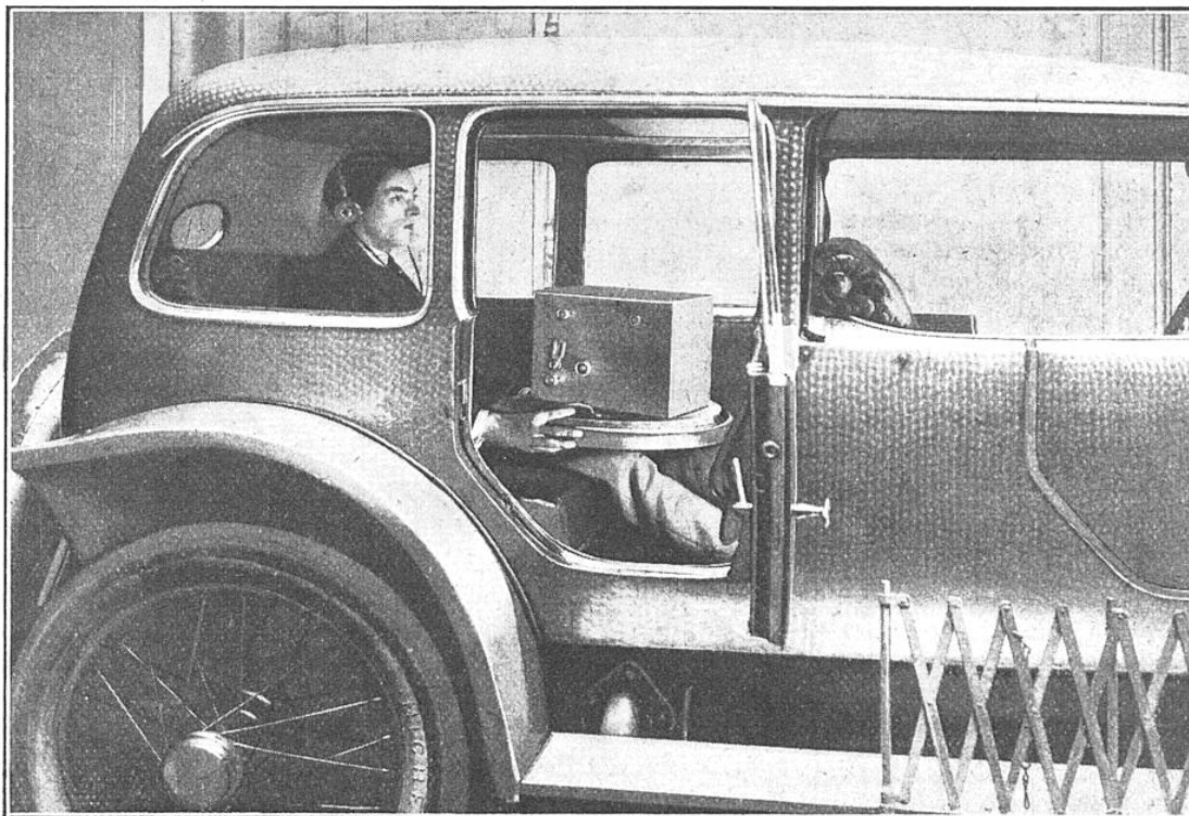
CETTE AUTOMOBILE CONTIENT LE MICRORADIOGONIOMÈTRE, QUI PERMET DE SITUER EXACTEMENT, DANS L'ESPACE DÉLIMITÉ PAR LES RECOUPEMENTS OBTENUS AVEC LES POSTES FIXES, L'ENDROIT OU SE TROUVE LE POSTE CLANDESTIN
