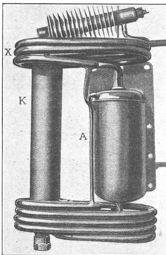
FIG. 1. — L'APPAREIL PLATEN-MUNTERS A, absorbeur ; K, bouilleur ; X, refroidisseur.
