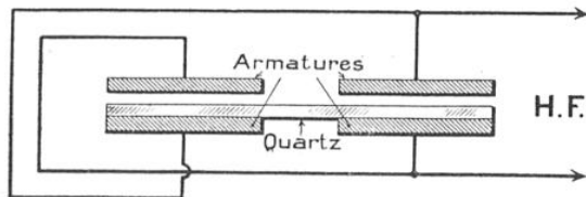
FIG. 7. — DISPOSITIF PERMETTANT L'OBSERVATION D'HARMONIQUES PAIRS
