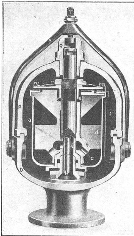
FIG. 2. — ÉPURATEUR D'HUILE CENTRIFUGE
