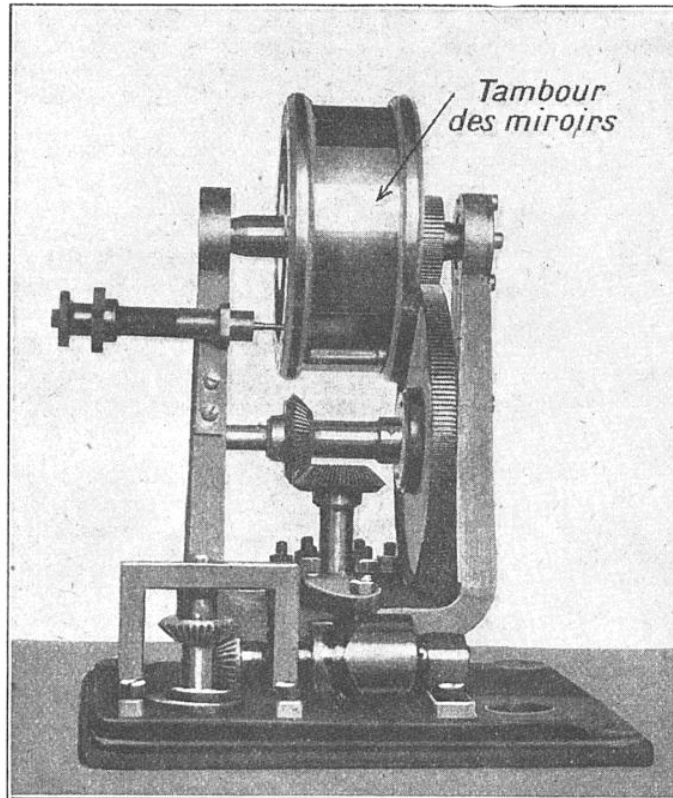
LE TAMBOUR DES MIROIRS SUR SON BÂTI, AVEC LES COMMANDES RÉALISANT LE MOUVEMENT DE ROTATION, COMBINÉ AVEC LE MOUVEMENT ALTERNATIF
