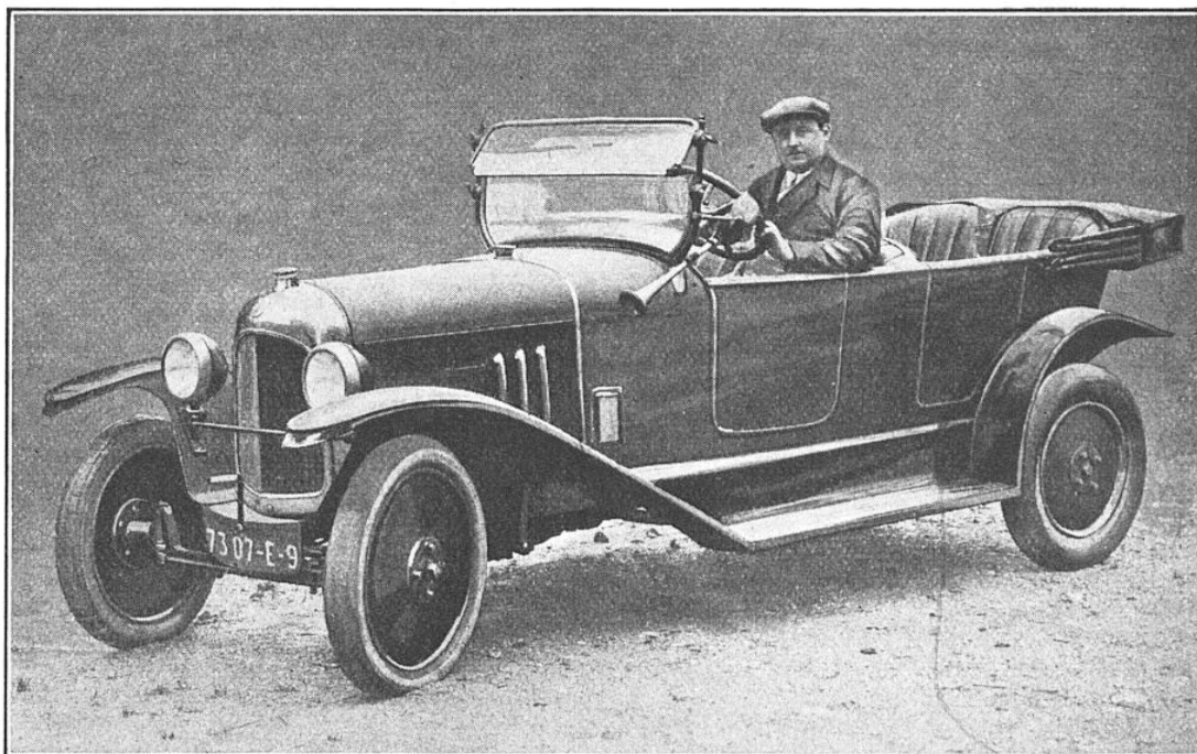
VOITURE 10 C. V. DE SÉRIE AYANT SERVI DEPUIS 1922 AUX EXPÉRIENCES DE M. DUMANOIS
