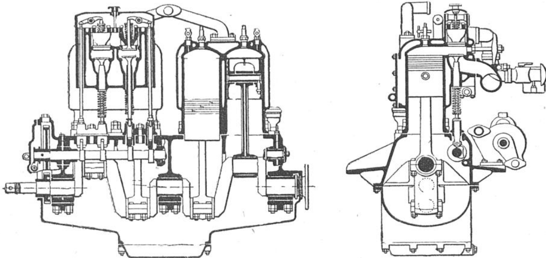
MOTEUR DE 60-80 C. V. MONTÉ SUR LES NOUVELLES AUTOMOTRICES
