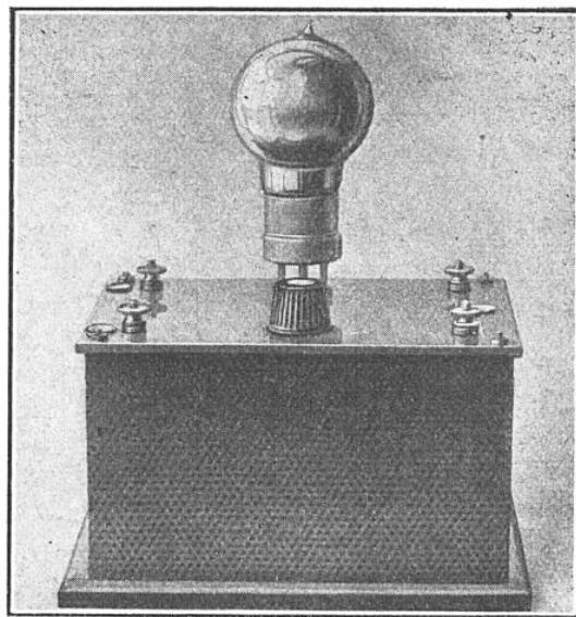
L'APPAREIL REDRESSEUR DE COURANT MUNI DE SA LAMPE SPÉCIALE
