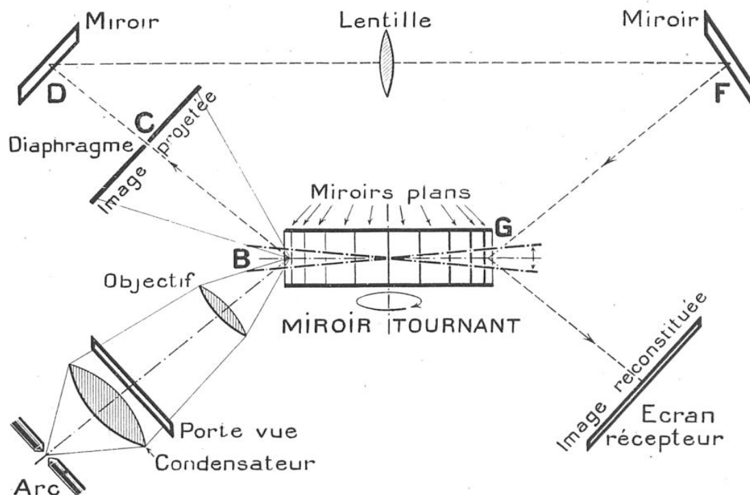
FIG. 3. — DESSIN SCHÉMATIQUE DE L'INSTALLATION REPRÉSENTÉE PAR LA PHOTOGRAPHIE DE LA PREMIÈRE PAGE
