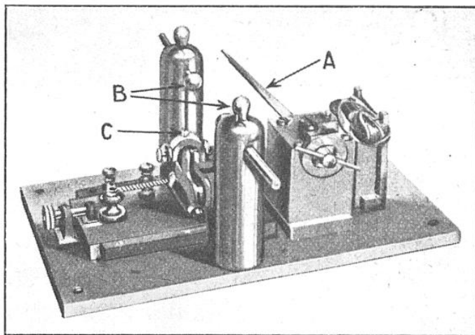
FIG. 7. — INTERRUPTEUR D'ÉTINCELLE
