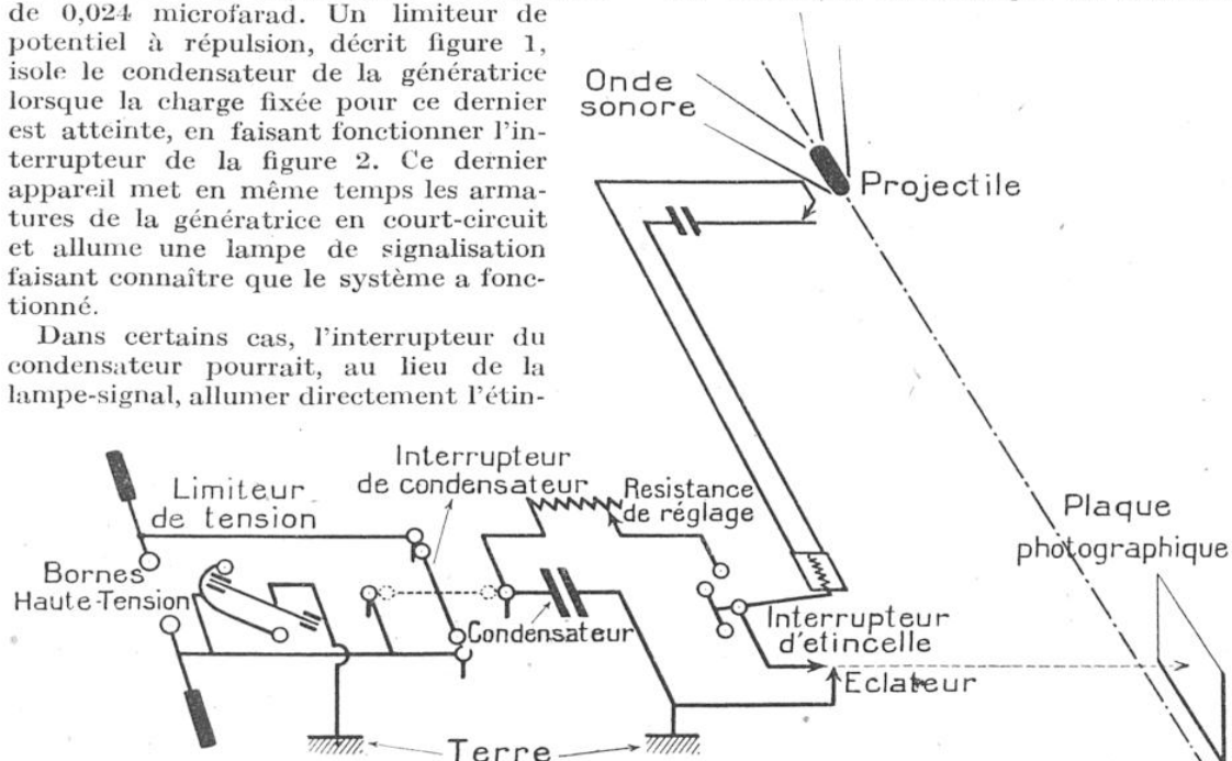
FIG. 4. — SCHÉMA DU DISPOSITIF DE PHOTOGRAPHIE AUTOMATIQUE DES PROJECTILES
