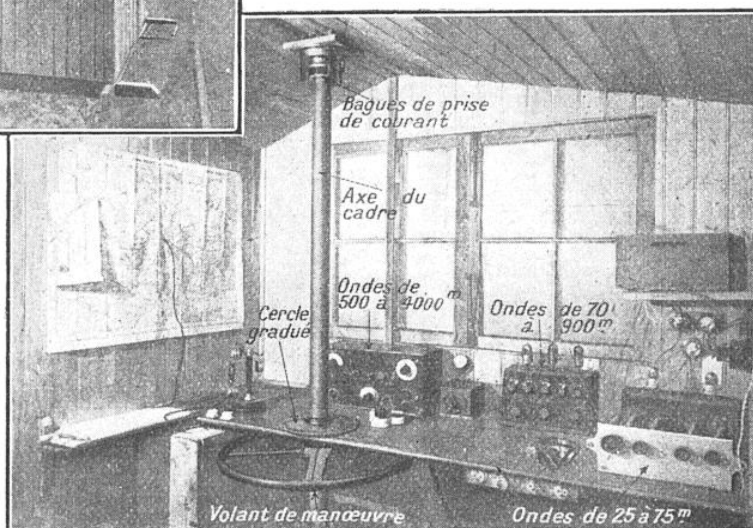
VUE INTÉRIEURE DU POSTE : APPAREILS DE RÉCEPTION
