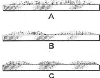
FIG. 6. — DIVERS ASPECTS DE L'EFFLUVE SUR LE CRISTAL OSCILLANT
