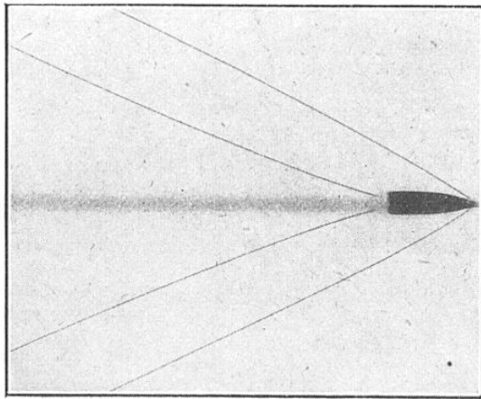
FIG. 5. — PHOTOGRAPHIE DU PASSAGE D'UNE BALLE DE REVOLVER DANS L'AIR
