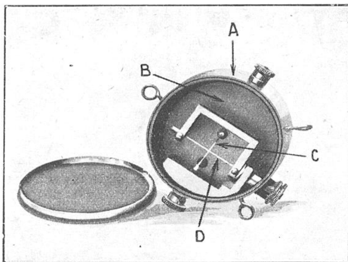
FIG. 3. — CONTACTEUR AUTOMATIQUE PAR CHOC SONORE
