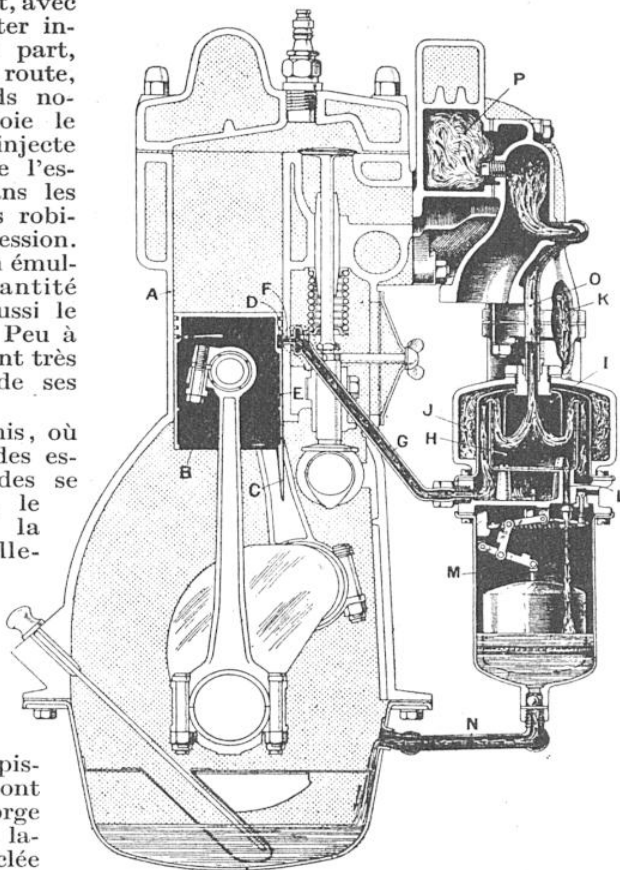
FIG. 3. — INSTALLATION D'UN SÉPARATEUR D'HUILE SUR UN MOTEUR
