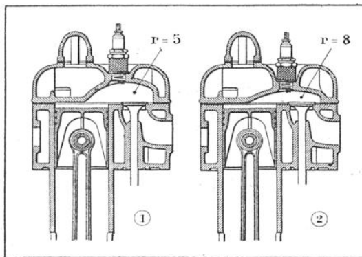
VARIATIONS DU RAPPORT DE COMPRESSION 1, conditions normales ; r , rapport volumétrique égal 5, maximum pratique ; 2, avec l'emploi des antidétonants, ce rapport peut être porté à 8.
