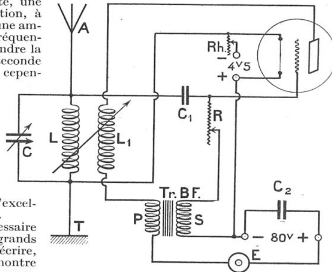
FIG. 4. — MONTAGE D'UNE DÉTECTRICE À RÉACTION AVEC CIRCUIT RÉFLEXE
