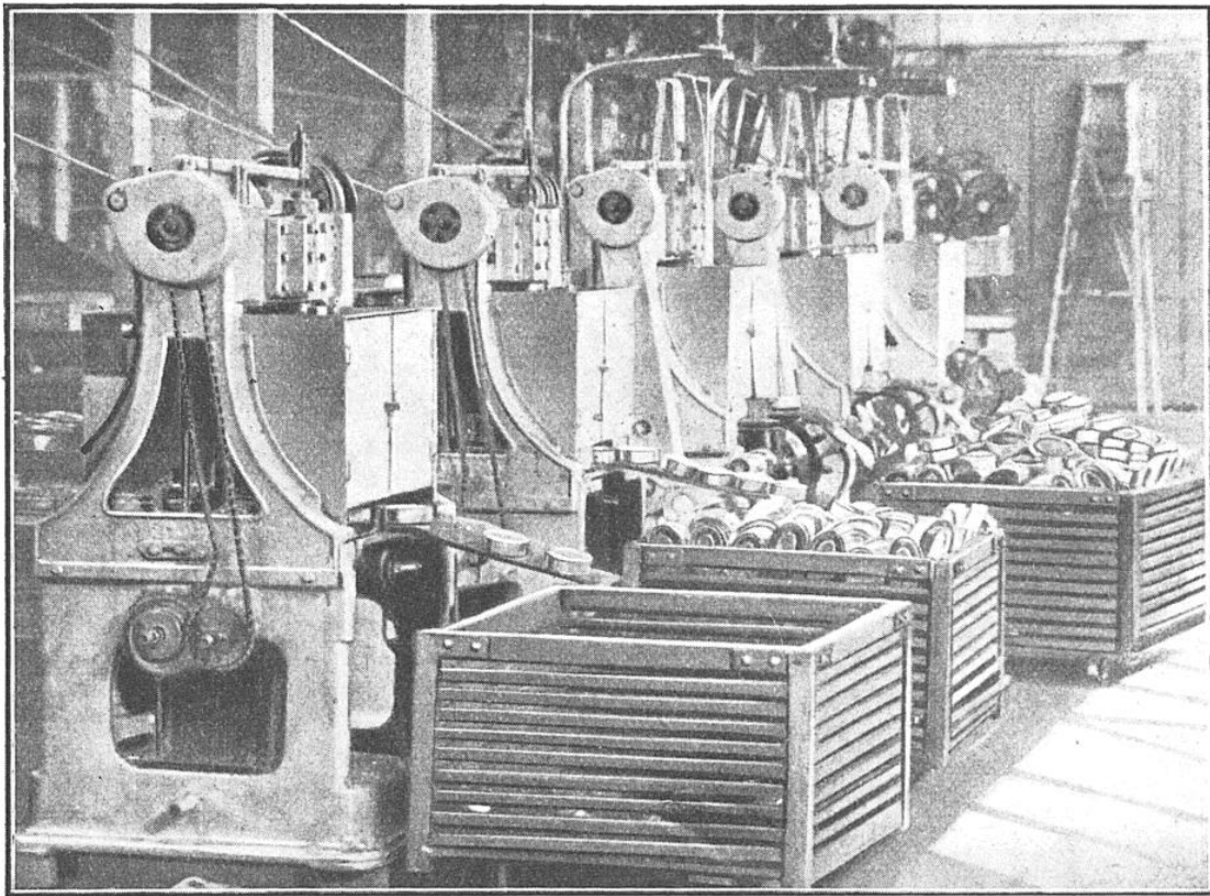
FIG. 7. — SERTISSAGE MÉCANIQUE DES BOÎTES, PRÉALABLEMENT GARNIES DE SARDINES
