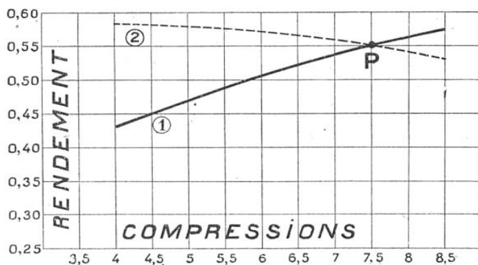
COURBES DES VARIATIONS DU RENDMENT D'UN MOTEUR AVEC LA COMPRESSION
