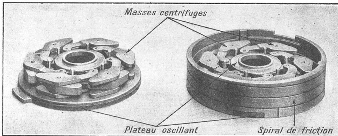
DIVERSES PIÈCES CONSTITUTIVES DE L'EMBRAYAGE FIEUX
