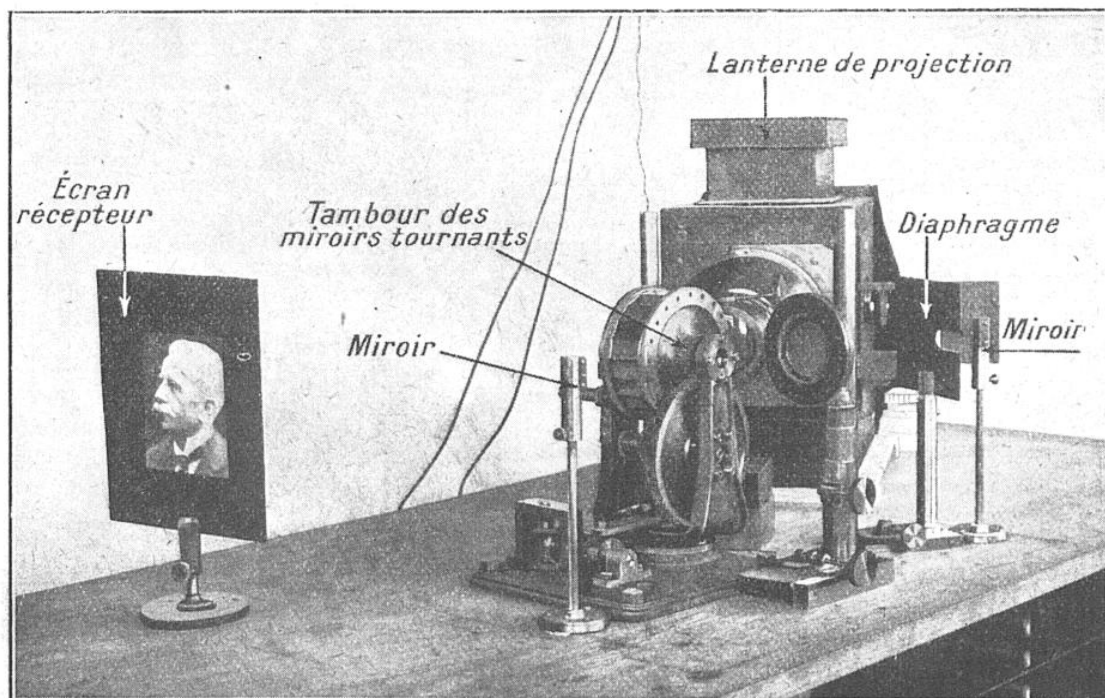
LE DERNIER APPAREIL D'EXPÉRIENCE DE M. ÉDOUARD BELIN
