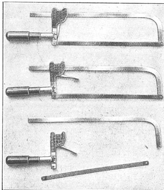
CETTE MONTURE DE SCIE PERMET D'UTILISER DES LAMES DE LONGUEURS DIVERSES
