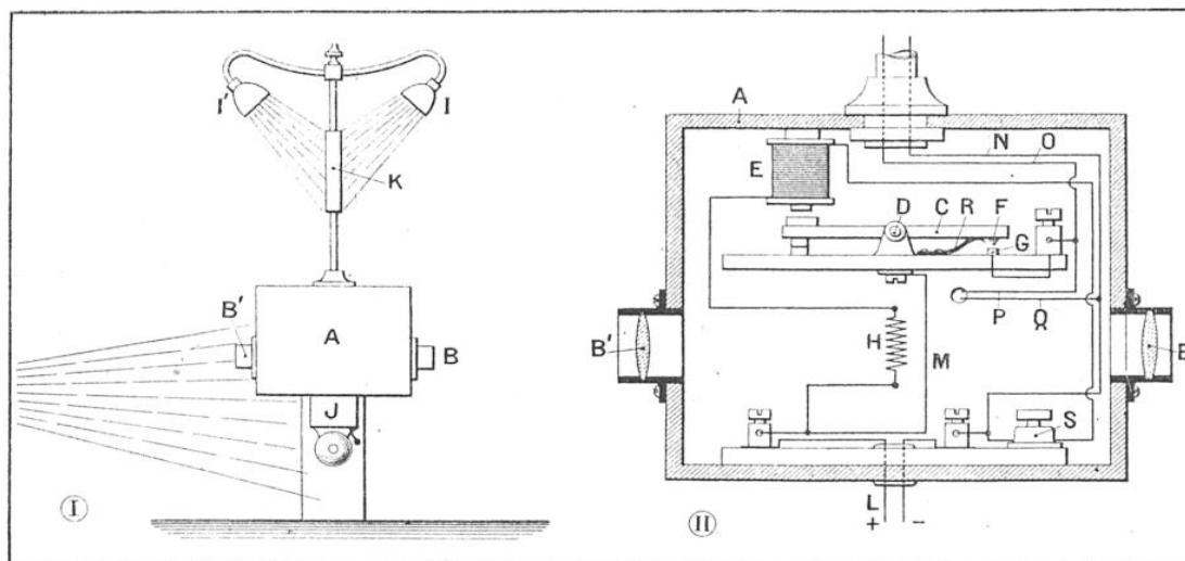
FIG. 5. — AVERTISSEUR NOCTURNE A FONCTIONNEMENT AUTOMATIQUE
