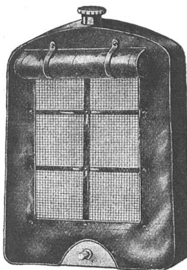
FIG. 6. — COUVRE-RADIATEUR AJUSTÉ SUR LA CALANDRE ET PORTANT UN RIDEAU MOBILE PERMETTANT DE MASQUER LE RADIATEUR
