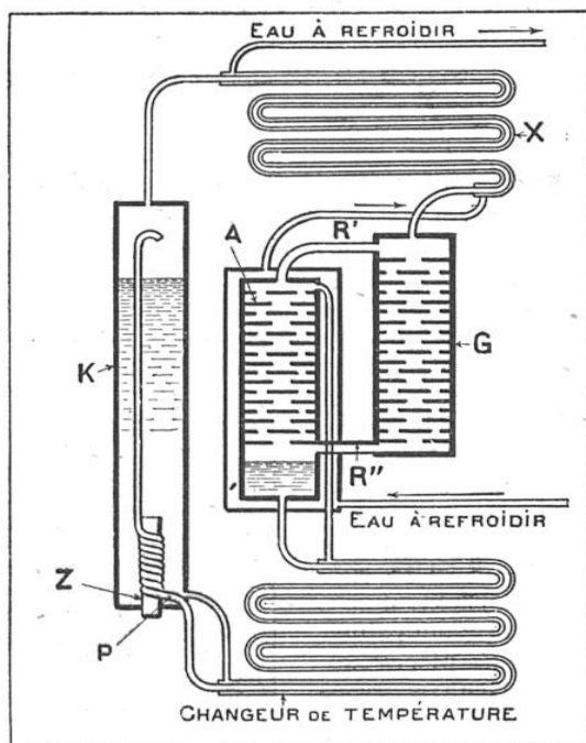
FIG. 2. — SCHÉMA DU FONCTIONNEMENT DE LA NOUVELLE MACHINE PLATEN-MUNTERS K, bouilleur ; G, générateur ; X, refroidisseur ; Z, source de chaleur ; R', entrée de l'hydrogène dans le générateur ; R'', sortie du mélange des vapeurs d'ammoniaque et de l'hydrogène ; P, tuyau remplaçant la pompe dans la machine Carré.
