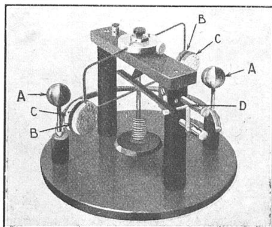
FIG. 1. — LIMITEUR DE POTENTIEL ÉLECTROSTATIQUE
