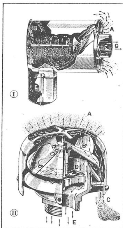
FIG. 1. — ÉPURATEURS D'AIR A MOUVEMENT GIRATOIRE
