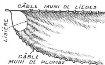
FIG. 3. — DÉTAIL DE L'EX- TRÉMITÉ D'UNE AILE
