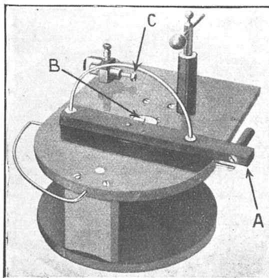
FIG. 2. — INTERRUPTEUR DE CHARGE DU CONDENSATEUR
