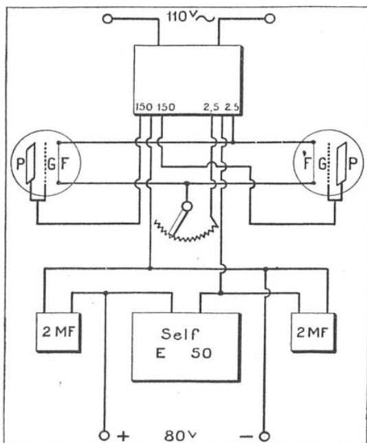
SCHEMA DU DISPOSITIF SUPPRIMANT LA BATTERIE DE TENSION DE PLAQUE
