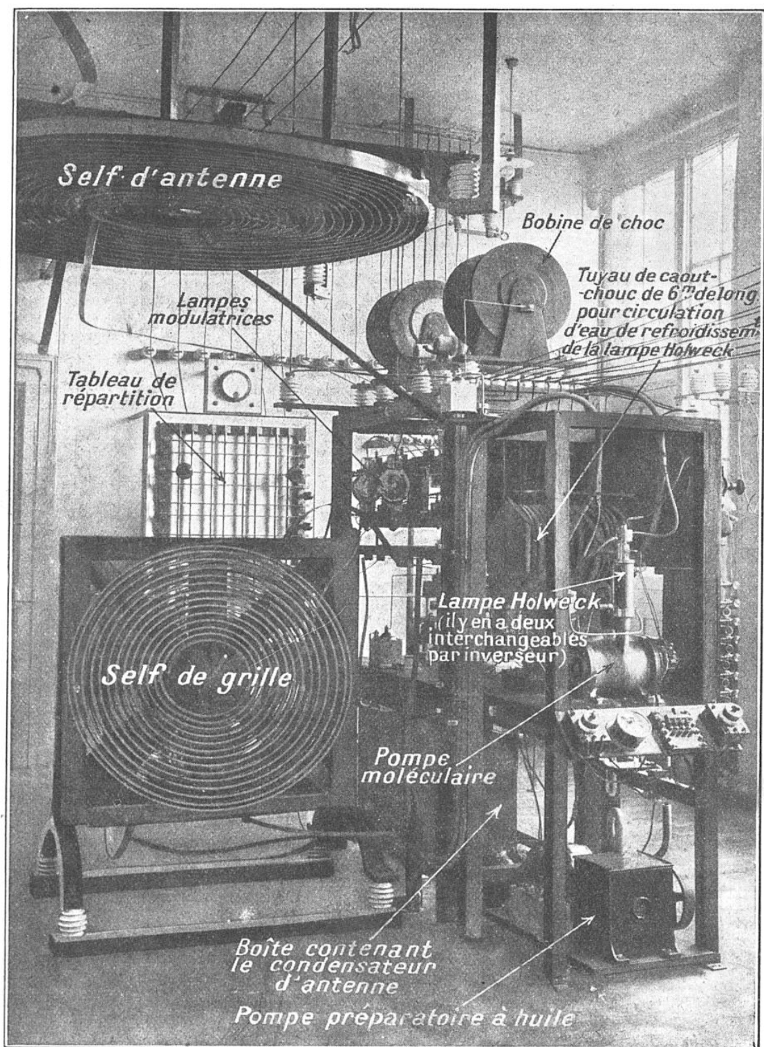
VUE INTÉRIEURE DU POSTE DE T. S. F. DE LA MALMAISON, A L'AIDE DUQUEL S'EFFECTUENT LES TRANSMISSIONS DE RADIOVISION
