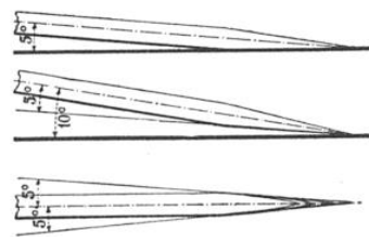
SCHEMA DE L'USURE D'UNE LAME PAR SUITE DES AFFILAGES SUCCESSIFS
