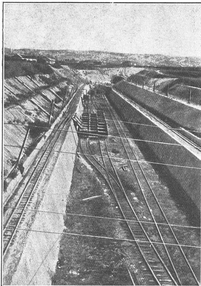
ÉTAT DES TRAVAUX, LE 5 SEPTEMBRE 1925, DE LA TRANCHÉE DE FOS, PRÈS DE PORT-DE-BOUC
