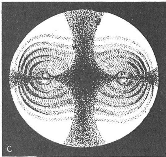
PLANCHE 2. — AUTRES ASPECTS D'UN CRISTAL DANS LE MICROSCOPE POLARISANT
