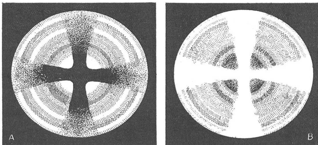
PLANCHE 1. — CE QUE L'ON VOIT DANS LE MICROSCOPE POLARISANT
