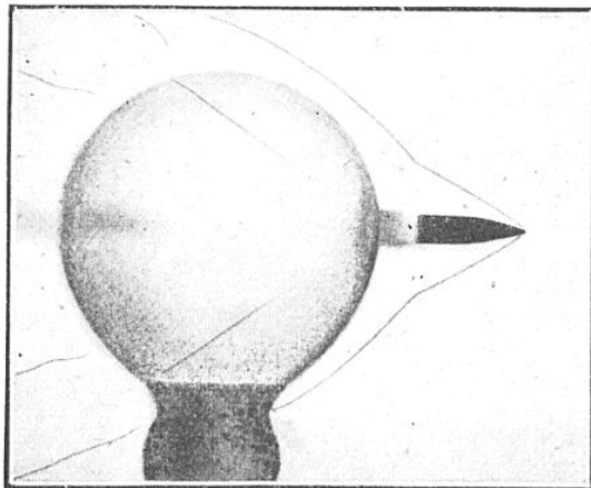
FIG. 6. — PASSAGE D'UNE BALLE A TRAVERS UNE BULLE DE SAVON GONFLÉE D'HYDROGÈNE On remarquera la déformation de la vague sonore produite par le passage du projectile dans des milieux de densités différentes.
