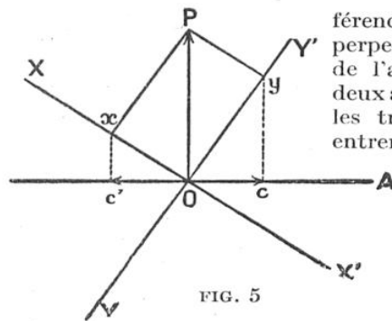
FIG. 5 DÉCOMPOSITION DES RAYONS LUMINEUX A TRAVERS UN CRISTAL ANISOTROPE
