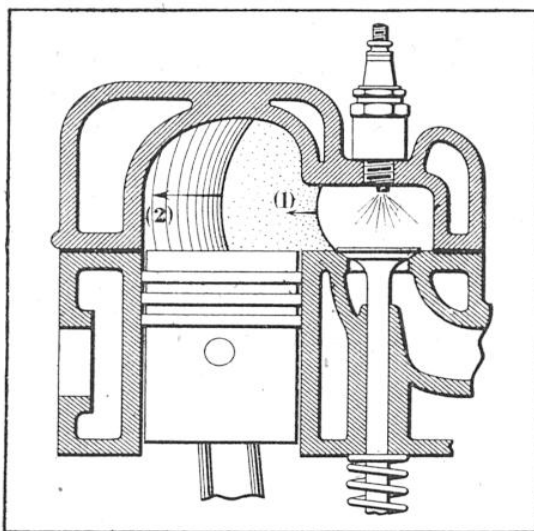
PROPAGATION DE L'EXPLOSION DANS UN MOTEUR
