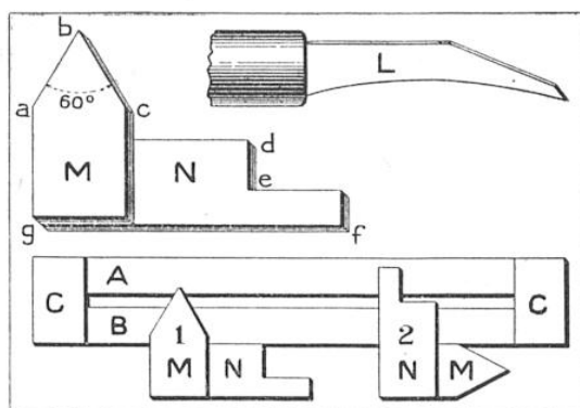
FIG. 3. — LES OUTILS DU GRAVEUR AMATEUR
