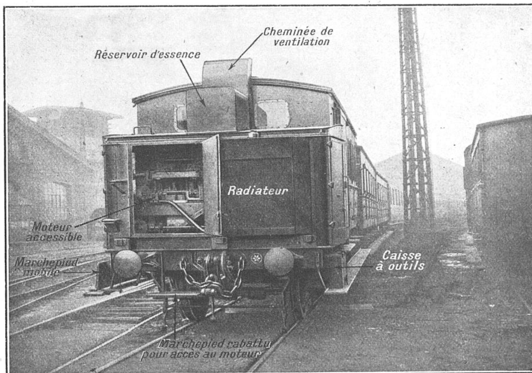
LA NOUVELLE AUTOMOTRICE A ESSENCE VUE DE L'AVANT
