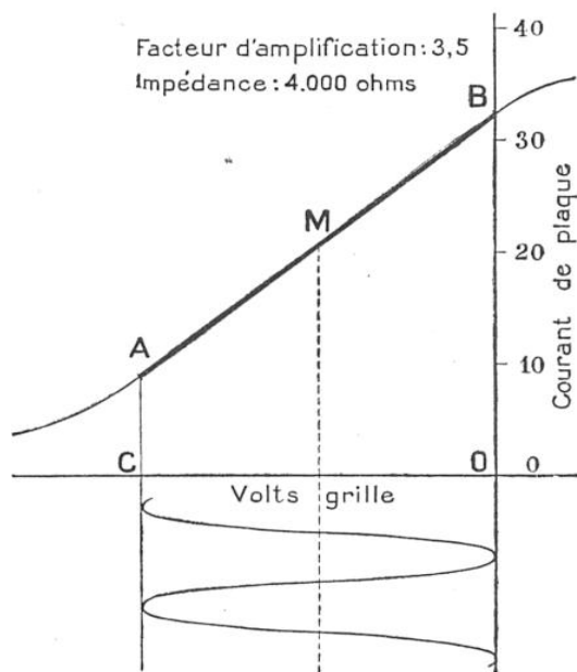
FIG. 2. — CARACTÉRISTIQUES D'UNE LAMPE A FAIBLE AMPLIFICATION
