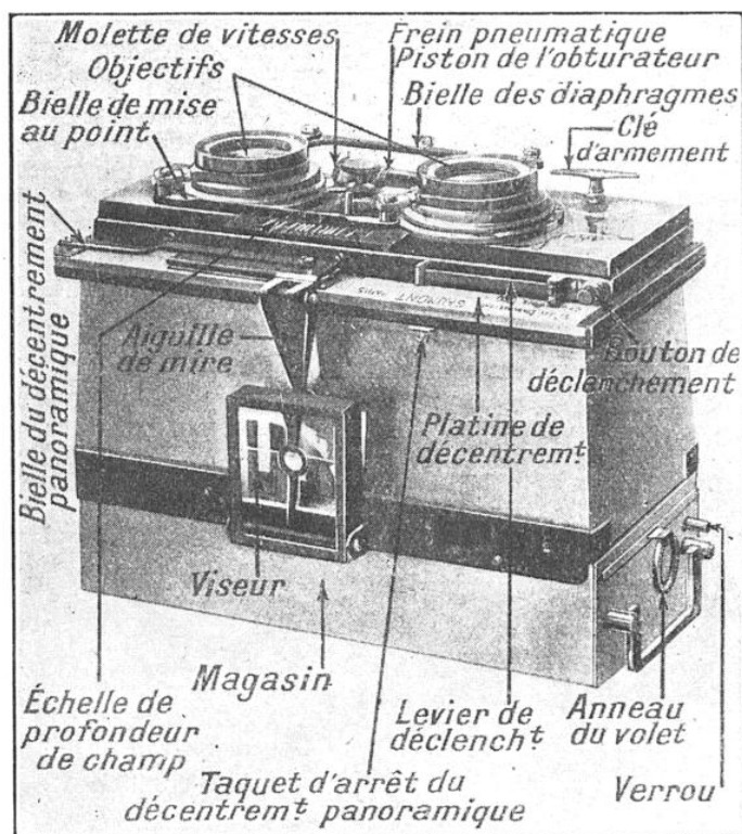
FIG. 26. — SPIDO MÉTALLIQUE GAUMONT
