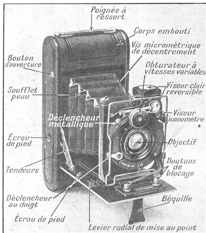
FIG. 20. - APPAREIL COCARETTE A PELLICULES
