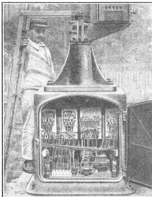
VUE D'UN RELAIS FRANÇAIS, A DEUX POSITIONS, COMMANDANT LES SIGNAUX
