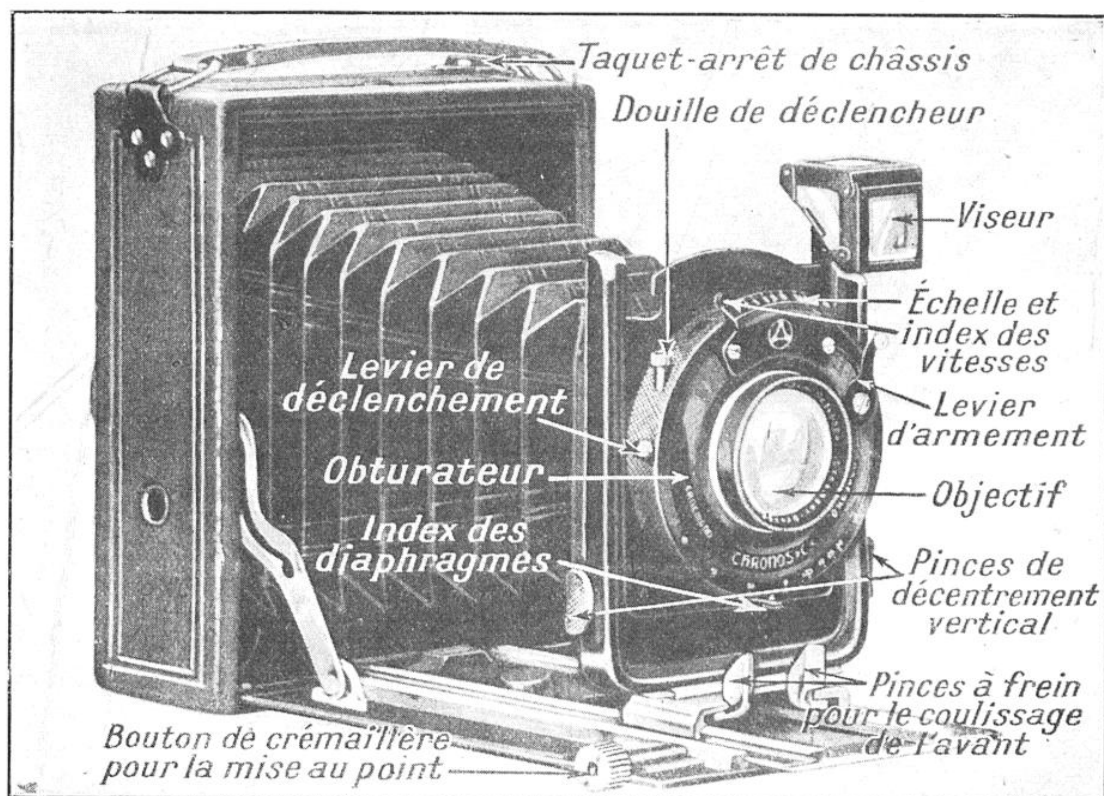
FIG. 7. — CHAMBRE « FOLDING » ERNEMANN
