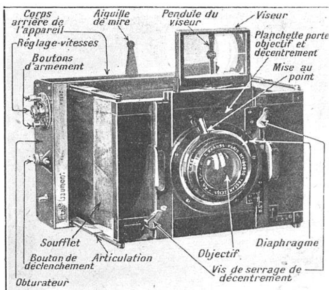
FIG. 14. — SPIDO PLIANT GAUMONT
