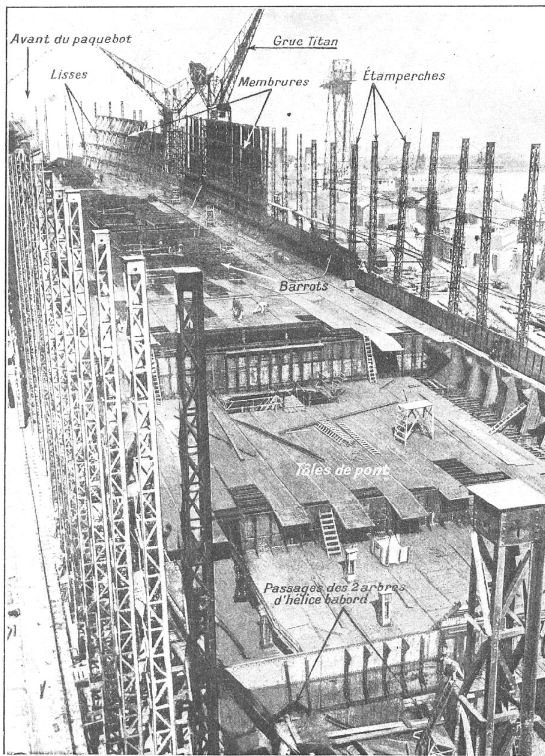
LE PAQUEBOT « ILE-DE-FRANCE » EN CONSTRUCTION A SAINT-NAZAIRE
