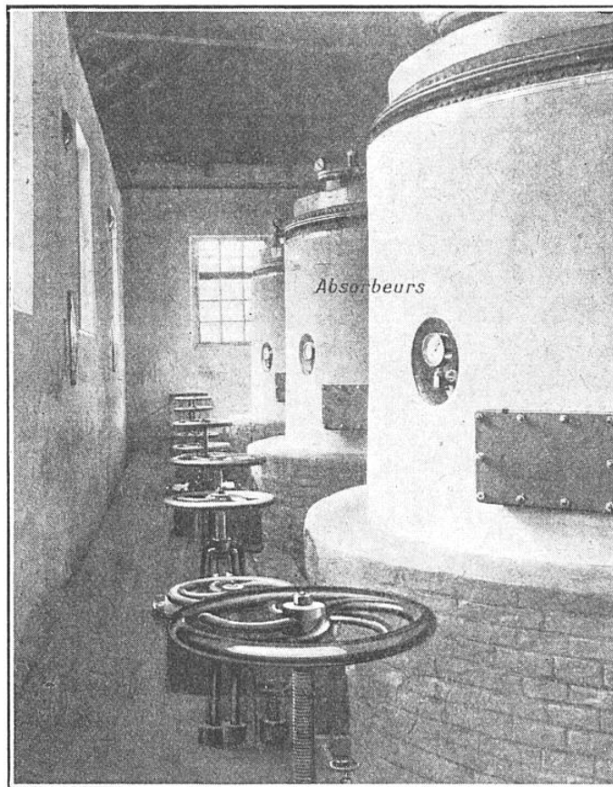
FIG. 8. — CETTE INSTALLATION REPRÉSENTE LES ABSORBEURS URBAIN UTILISÉS PAR UNE SOCIÉTÉ DE PÉTROLE DE BORYSLAW (POLOGNE)
