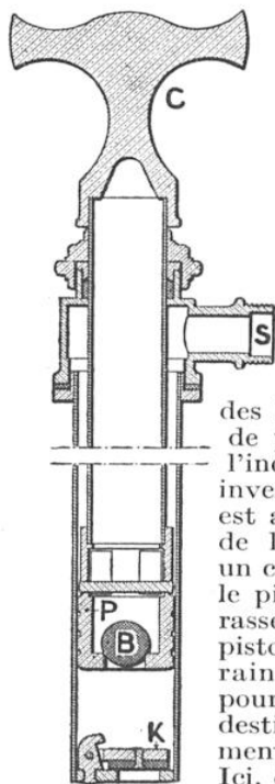
COUPE DE LA POMPE
