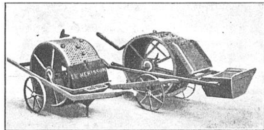
LE HÉRISSON, APPAREIL A RAMASSER LES POMMES A CIDRE
