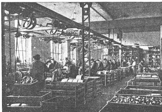
FABRICATION DES USTENSILES DE CUISINE EN ALUMINIUM Vue de l'atelier de repoussage à la manufacture de Tournus.
