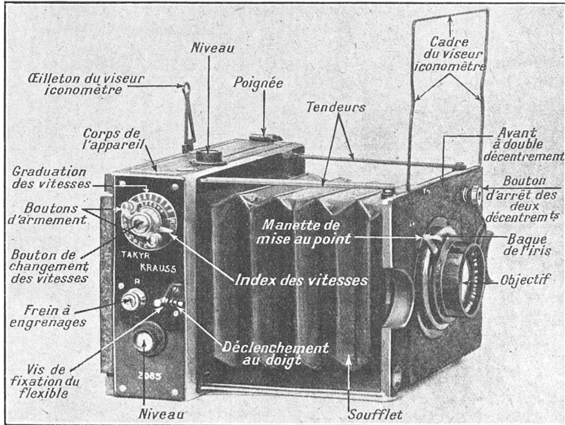
FIG. 12. — TAKYR-KRAUSS A OBTURATEUR DE PLAQUE
