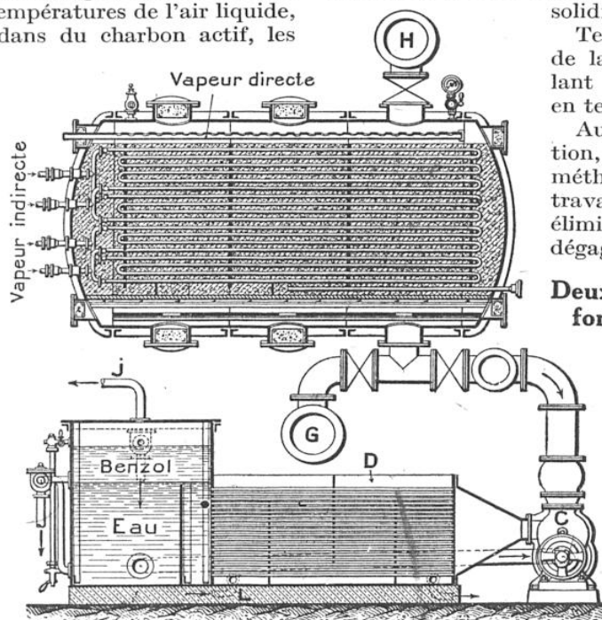
FIG. 9. — UNE INSTALLATION DESTINÉE A RÉCUPÉRER LE BENZOL CONTENU DANS LE GAZ D'ÉCLAIRAGE
