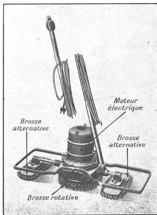
LA CIREUSE LA SEULE
