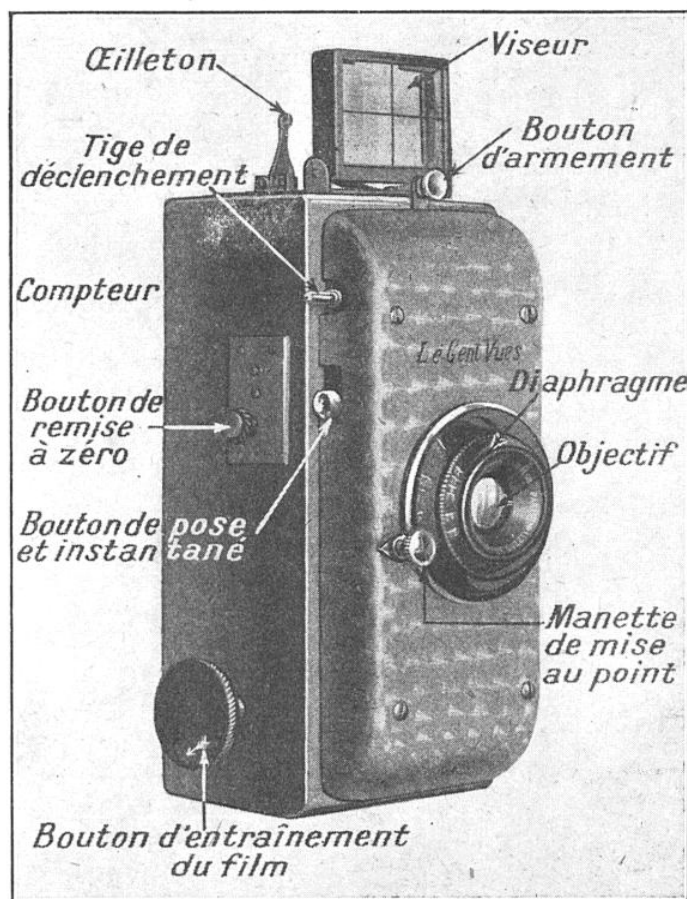
FIG. 28. — LE CENT VUES, APPAREIL A FILM
