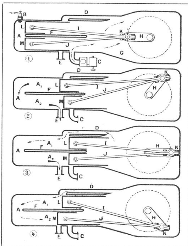
FIG. 3. — COUPES SCHÉMATIQUES D'UN MOTEUR LEYLAND A GROUPES DE DEUX CYLINDRES PARALLÈLES POSSÉDANT UNE CHAMBRE D'EXPLOSION COMMUNE
