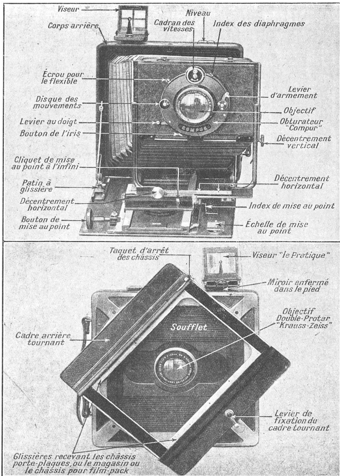
FIG. 13. — ACTIS KRAUSS. CHAMBRE FOLDING, AVEC CADRE ARRIÈRE TOURNANT
