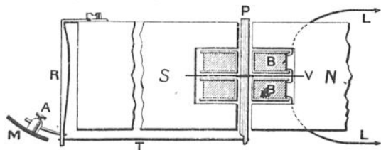
FIG. 7. — LE « MOTEUR » DU HAUT-PARLEUR ET SA LIAISON AVEC LA MEMBRANE VIBRANTE
