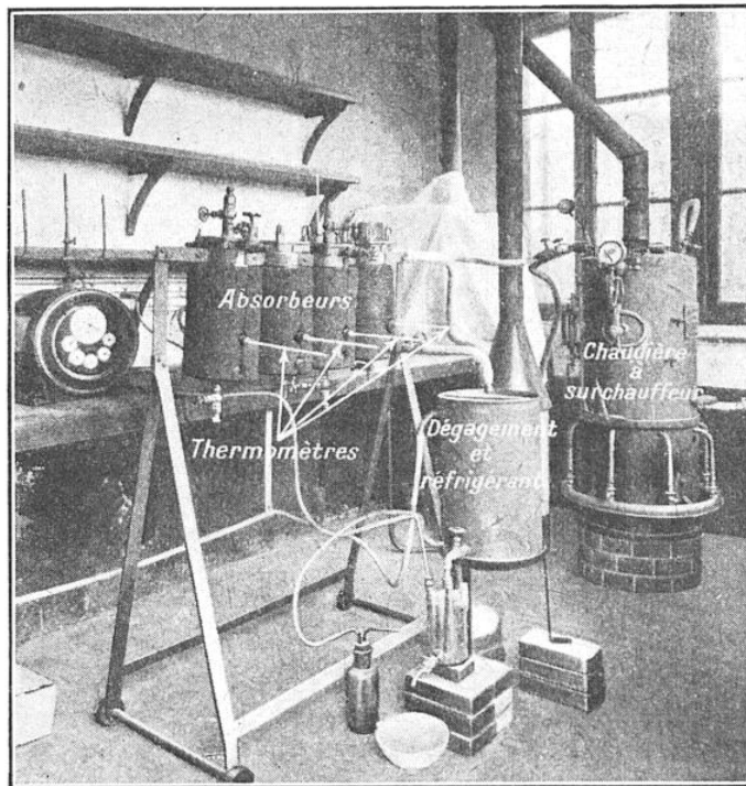
FIG. 10. — EXPÉRIENCE IMPORTANTE DE M. SABRON, INGÉNIEUR DE LA SOCIÉTÉ DU GAZ DE PARIS, METTANT EN RELIEF L'EFFICACITÉ DE LA VAPEUR D'EAU POUR L'EXTRACTION DES GAZ ABSORBÉS
