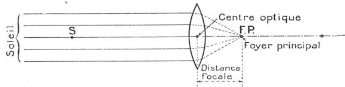
FIG. 5. — QUELQUES CARACTÉRISTIQUES D'UNE LENTILLE
