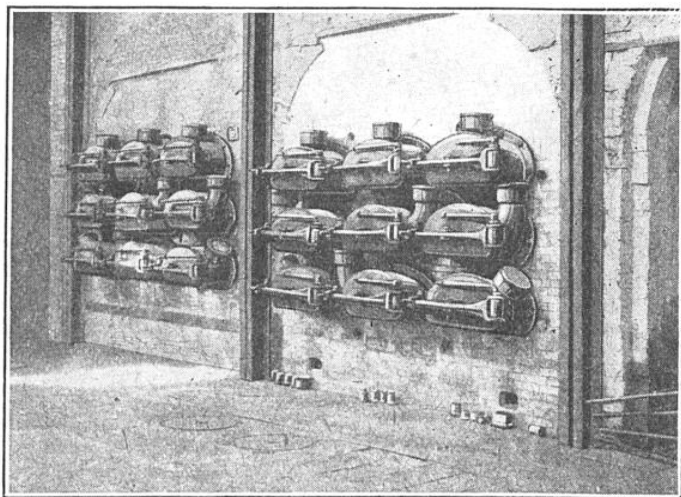
FIG. 3. — BATTERIES DE FOURS, À L'USINE DE NANTERRE (SEINE), DANS LESQUELLES ON ACTIVE LE CHARBON DE TOURBE SUIVANT LE PROCÉDÉ ÉDOUARD URBAIN
