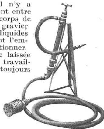
VUE DE LA POMPE MONTÉE SUR UN TRÉPIED
