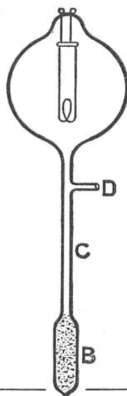
FIG. 7. - LE VIDE PEUT ÊTRE OBTENU PAR LE CHARBON
