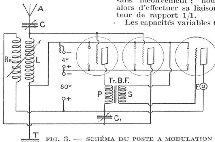
FIG. 3. — SCHÉMA DU POSTE A MODULATION
