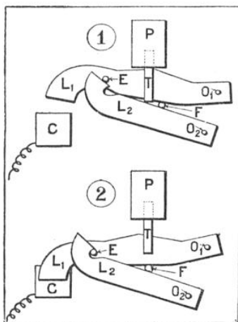
SCHÉMA DE FONCTIONNEMENT DU BOUTON-POUSOIR
