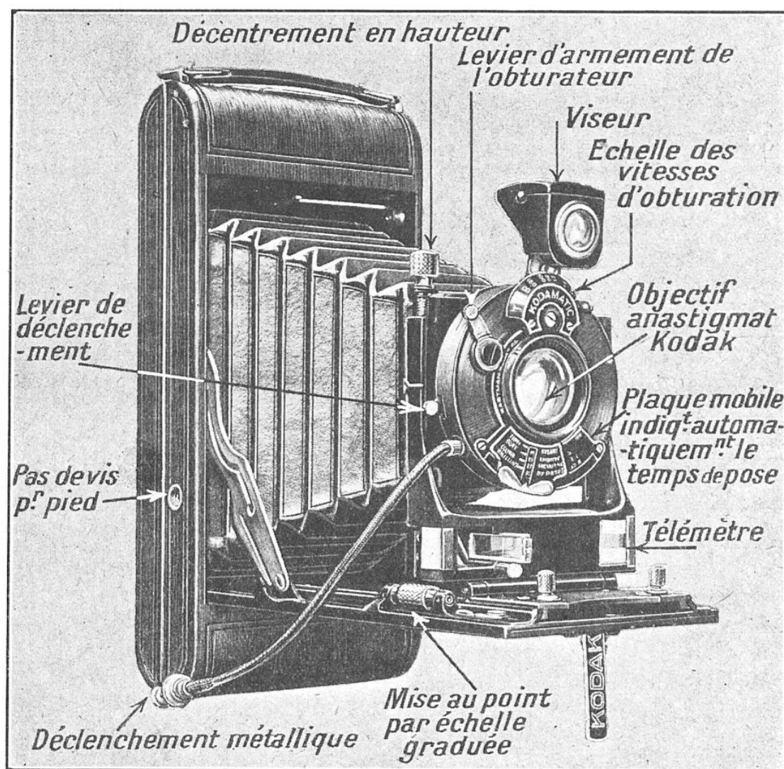
FIG. 19. — « KODAK SPÉCIAL » AUTOGRAPHIQUE
