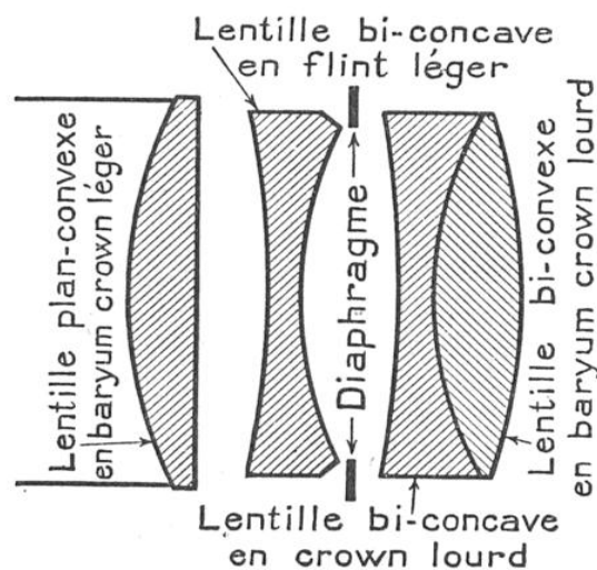
FIG. 18. — OBJECTIF TESSAR ZEISS-KRAUSS
