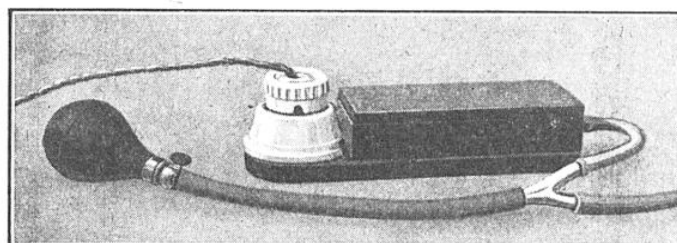
GRACE A CET APPAREIL, UNE PRESSION EXERCÉE SUR LA POIRE DE CAOUTCHOUC ASSURE EN MÊME TEMPS L'OUVERTURE DE L'OBTURATEUR ET L'INFLAMMATION DE LA POUDRE ÉCLAIRANTE
