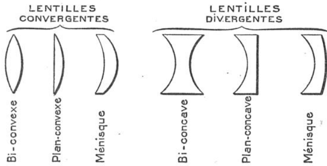
FIG. 8. — LENTILLES EMPLOYÉES DANS LES OBJECTIFS
