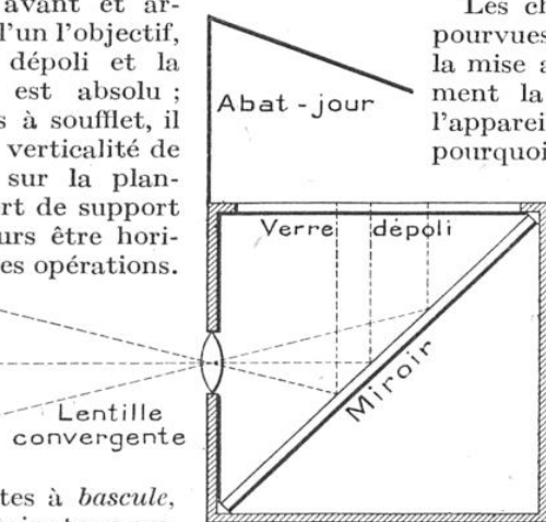
FIG. 16. — UN VISEUR
