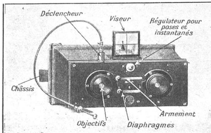
FIG. 25. — JUMELLE STÉRÉOSCOPIQUE « CAPSA »
