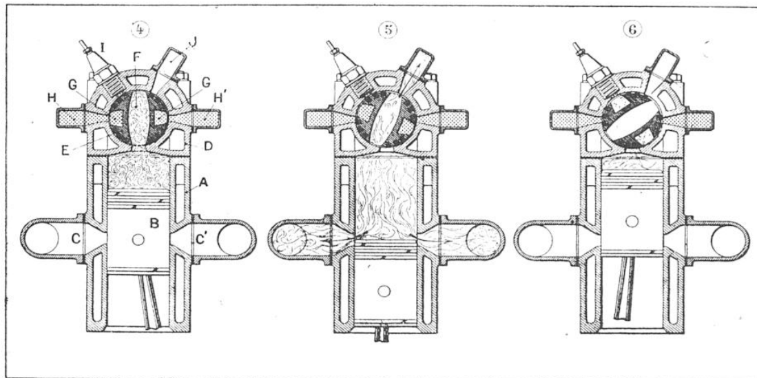
FIG. 5. — LE MOTEUR MICHEL WOLFF A DEUX TEMPS ET PHASES DU CYCLE MATHÉMATIQUEMENT SÉPARÉES
