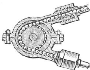
DANS CETTE TRANSMISSION, L'EFFORT EST TRANSMIS PAR DES FILES DE BILLES D'ACIER
