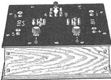
"RECTIFILTRE" plaque pour alternatif.
