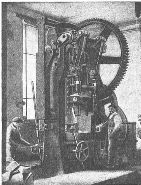
UNE PHASE DE LA FABRICATION DES USTENSILES EN ALUMINIUM
