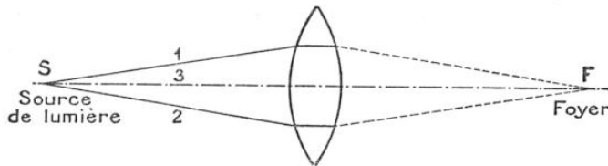
FIG. 4. — MARCHÉ DES RAYONS LUMINEUX A TRAVERS UNE LENTILLE
