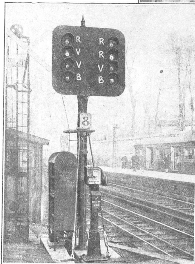
DÉTAIL D'UN SIGNAL LUMINEUX, SYSTÈME AMÉRICAIN, DE LA GARE DE MEUDON-VAL-FLEURY
