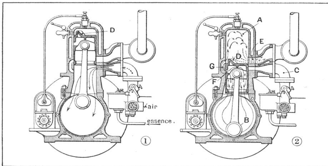
FIG. 2. — COUPES D'UN MOTEUR SANS SOUPAPES A DEUX TEMPS, DONT LE CARTER INFÉRIEUR SERT DE CORPS DE POMPE D'ALIMENTATION
