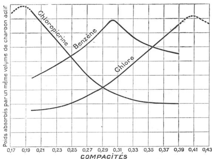
FIG. 6. — CE GRAPHIQUE MONTRE COMMENT VARIE LA FACULTÉ D'ABSORPTION D'UN CHARBON AVEC DES CORPS DIFFÉRENTS
