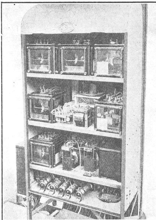
ENSEMBLE DES RELAIS AMÉRICAIN SITUÉS AU PIED D UN SIGNAL
