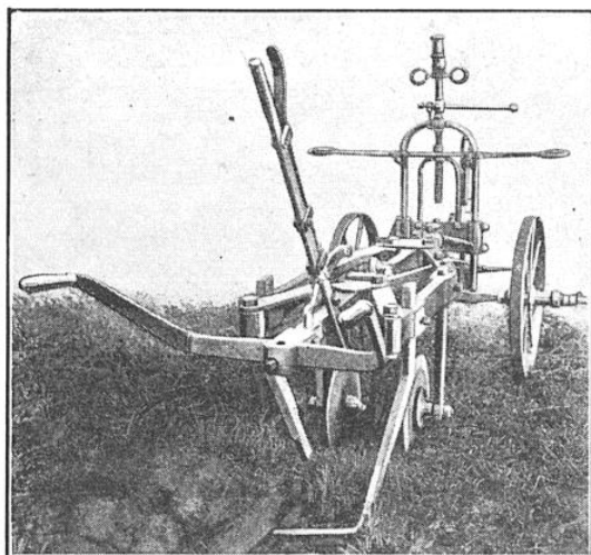
CHARRUE BAJAC A OUVRIR LES RIGOLLES DANS LES PRAIRIES
