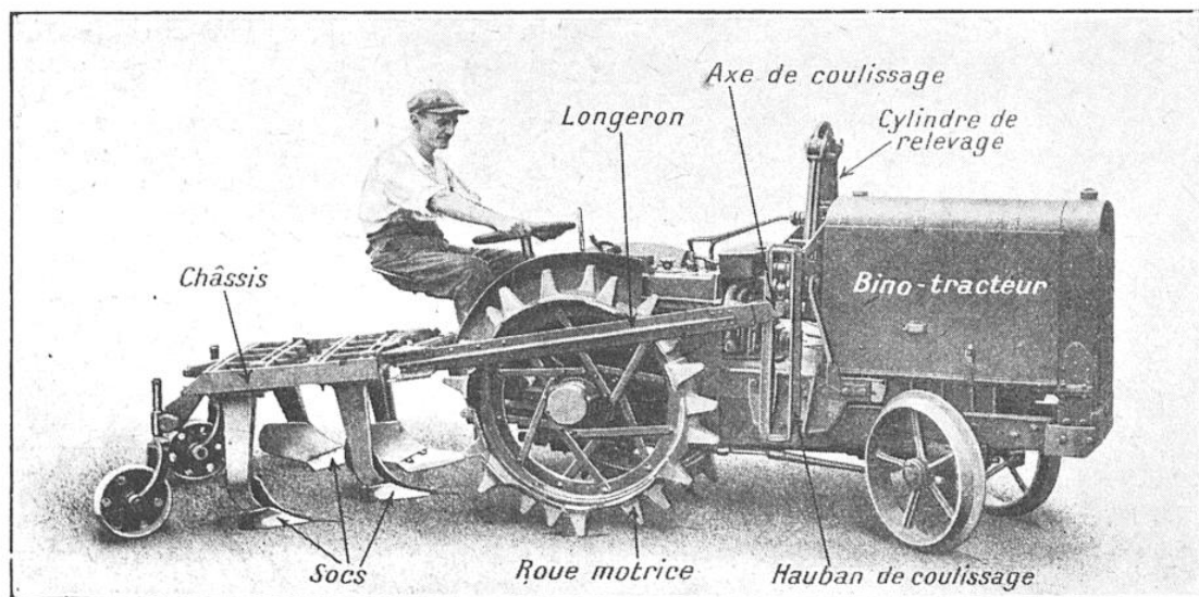
BINO-TRACTEUR BAUCHE, MODÈLE VIGNERON
