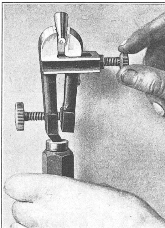
CETTE PHOTOGRAPHIE MONTRE NETTEMENT QU'UNE PIÈCE CONIQUE EST TRÈS BIEN SERRÉE PAR CET ÉTAU
