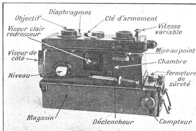
FIG. 27. — LE VÉRASCOPE RICHARD
