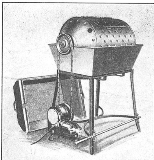
MACHINE « BIRUM » A LAVER LE LINGE
