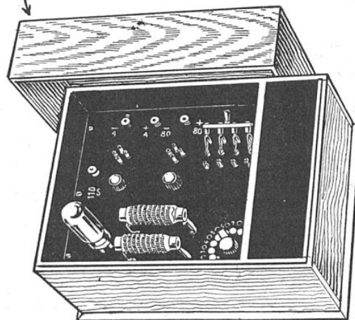
"RECTIFILTRE UNIVERSEL" 4 et 80 V.
