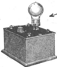
"REDRESSEUR-FILTRE" avec lampe biplaque redres- sant les 2 1/2 périodes pour toute tension de 30 à 250 V.
