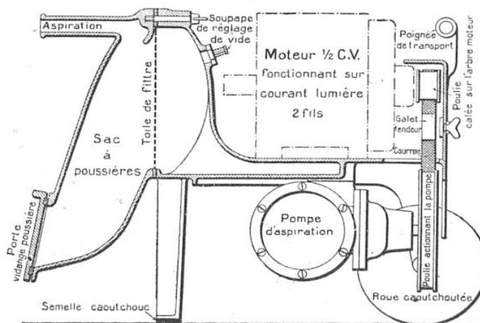
VUE EN COUPE DE L'ASPIRATEUR SPIROS
