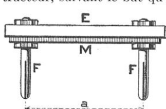
FIG. 4. — FICHE DOUBLE DE DISTRIBUTION
