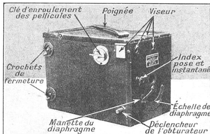
FIG. 1. — APPAREIL DÉTECTIVE PHOTO-HALL POUR DÉBUTANTS, A PELLICULE OU A PLAQUES
