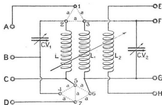
FIG. 5. — SCHÉMA DE LA BOÎTE D'ACCORD UNIVERSELLE
