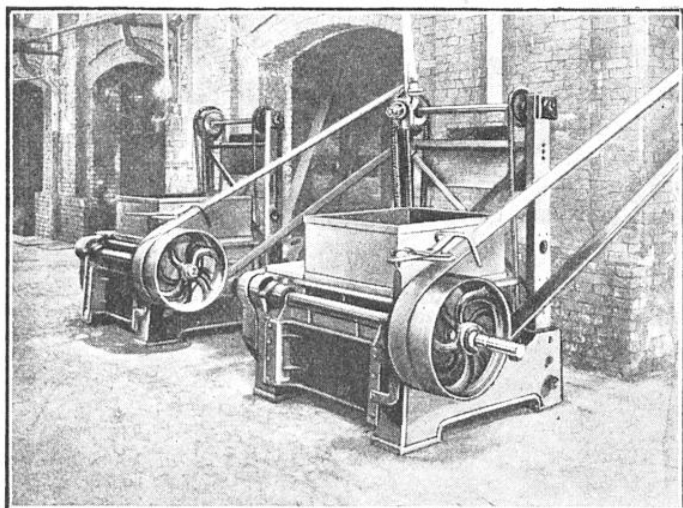
FIG. 2. — MALAXEURS SERVANT À PRÉPARER LA TOURBE QUI, CARBONISÉE SUIVANT LE PROCÉDÉ URBAIN, FOURNIRA LE CHARBON ACTIF
