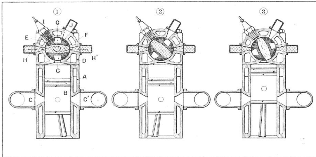
FIG. 4. — LE MOTEUR MICHEL WOLFF A DEUX TEMPS ET PHASES DU CYCLE MATHÉMATIQUEMENT SÉPARÉES
