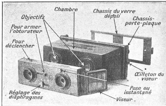
FIG. 23. — LE GLYPHOSCOPE, APPAREIL STÉRÉOSCOPIQUE POUR LES DÉBUTANTS
