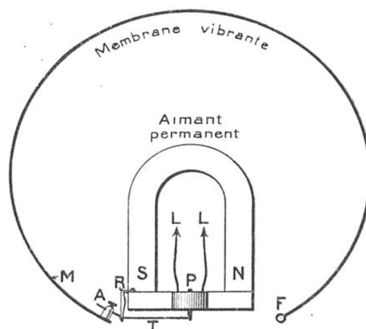
FIG. 6. — SECTION SCHÉMATISÉE DE L'AUDALION AU NIVEAU DU MOTEUR
