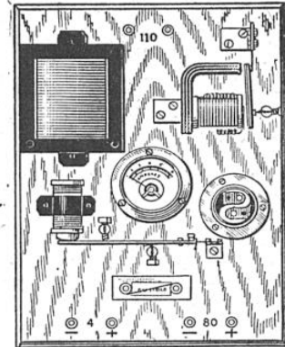
"TABLEAU A VIBREUR" 4 et 80 V. 4 A.
