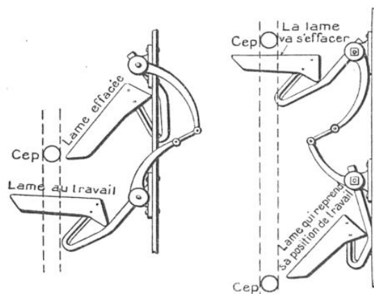
APPAREIL INTERCEPS LE « PHYLON »
