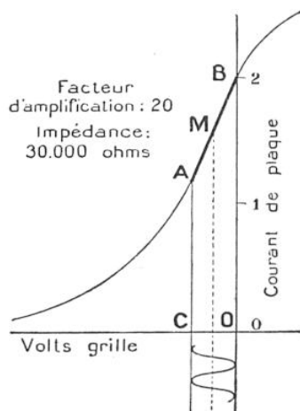
FIG. 1. — EXEMPLE DE CARACTÉRISTIQUES DE LAMPES A FORTE AMPLIFICATION
