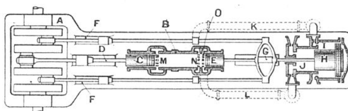
FIG. 1. — L'UN DES PREMIERS MOTEURS A DEUX TEMPS MUNI D'UN COMPRESSEUR SÉPARÉ D'ALIMENTATION : LE MOTEUR INDUSTRIEL OECHELHAUSER
