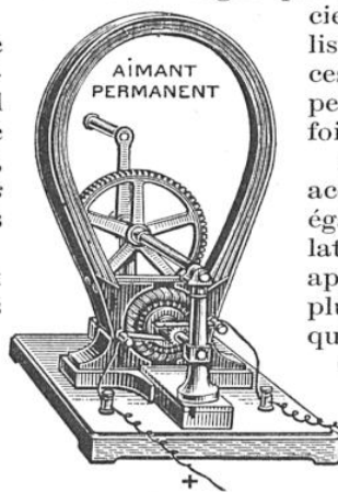
LA PREMIÈRE DYNAMO GRAMME
