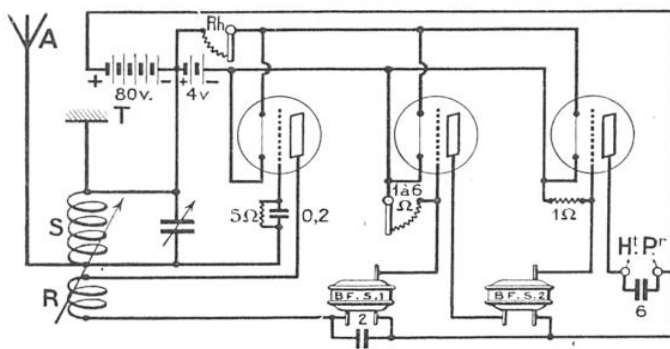
MONTAGE DU SURVOLTEUR DANS UN POSTE RÉCEPTEUR
