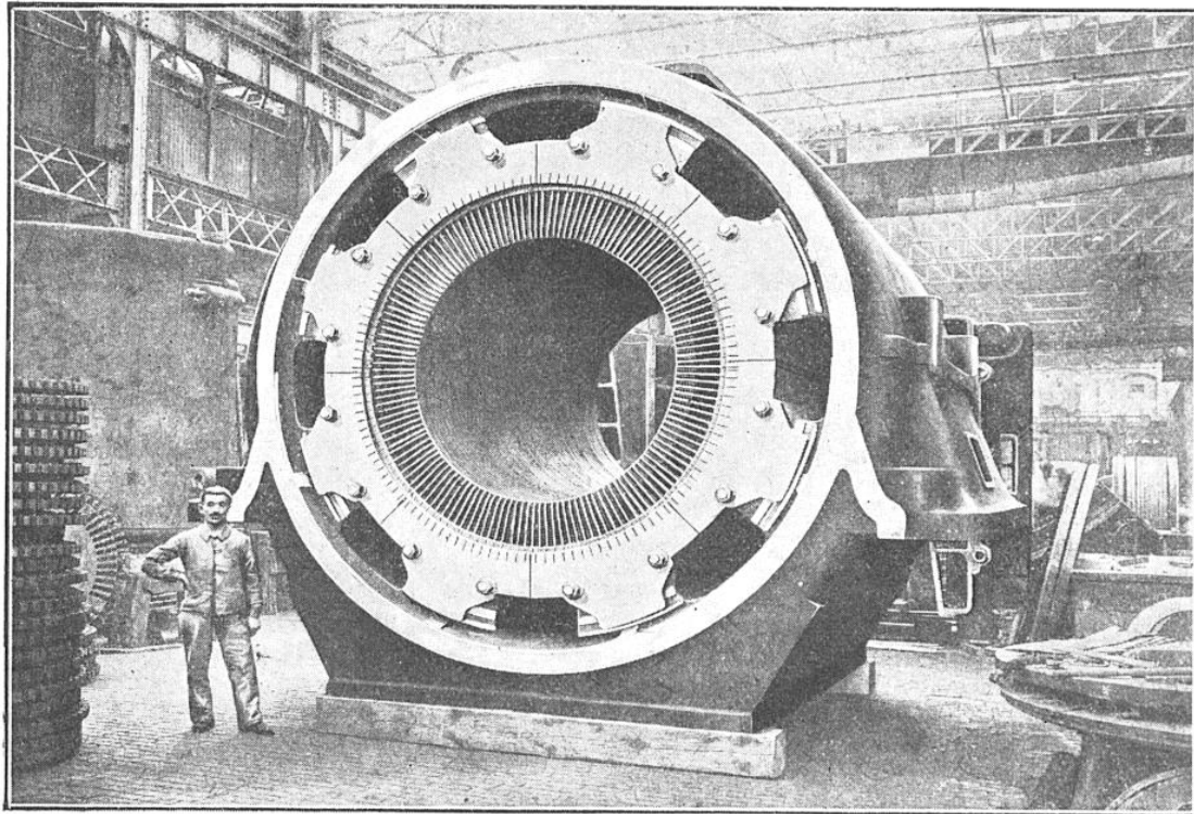
LE STATOR D'UN ALTERNATEUR DE 40.000 KILOWATTS DE LA CENTRALE DE GENNEVILLIERS Que de chemin parcouru en moins d'un siècle !... Les machines électriques modernes atteignent des dimensions considérables, et, cependant, aucun espace n'y est perdu pour la production de l'énergie.
