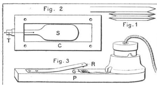
DÉTAIL DE L'APPAREIL CI-DESSUS
