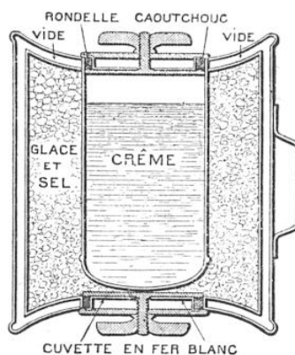
LA SORBETIÈRE PRESTO
