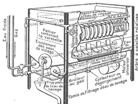
LA SIRÈNE, MACHINE À LAVER LA VAISSELLE C'est un appareil à grand débit.
