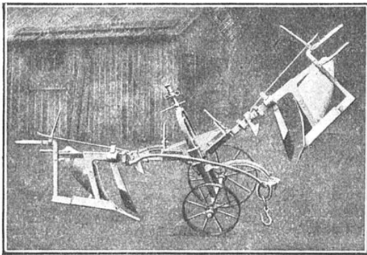
DÉFONCEUSE DOUBLE DELAHAYE
