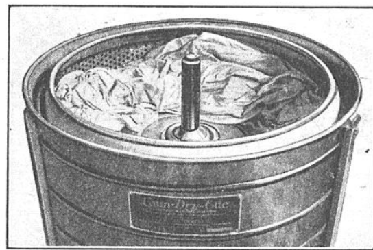
LA MACHINE AMÉRICAINE A LAVER LE LINGE Position du panier à linge pendant l'essorage.
