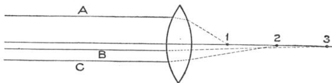
FIG. 6. — LES FOYERS DES RAYONS LUMINEUX NE SONT PAS TOUS AU MÊME POINT (LES DISTANCES 1, 2, 3 ONT ÉTÉ FORTEMENT EXAGÉRÉES)
