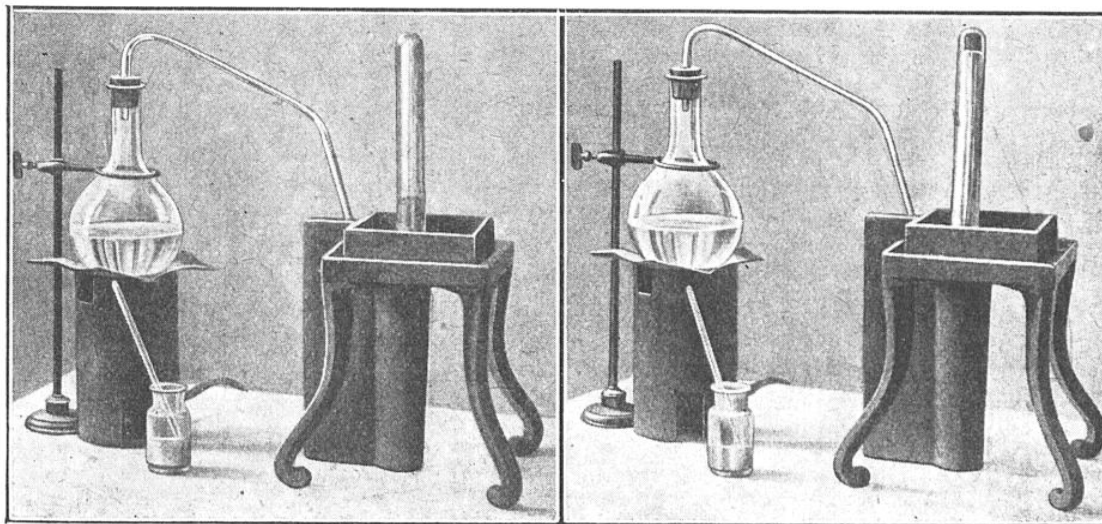
FIG. 1. — EXPÉRIENCE DE SAUSSURE MONTRANT LES PROPRIÉTÉS ABSORBANTES DU CHARBON A gauche : une éprouvette remplie, sur la cuve à mercure, de gaz ammoniac ; à droite : on introduit dans l'éprouvette un morceau de charbon de bois. Aussitôt le mercure remonte jusqu'au sommet de l'éprouvette. Le gaz semble avoir disparu. Il s'est, en réalité, totalement absorbé dans le charbon poreux.
