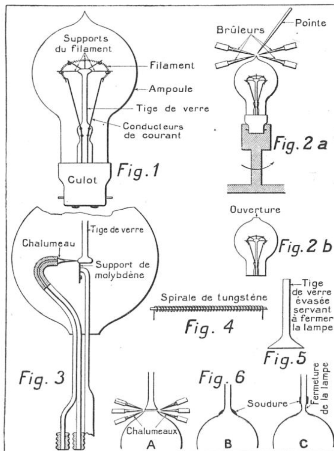
LES DIVERSES PHASES DE LA RÉGÉNÉRATION D'UNE LAMPE ÉLECTRIQUE À INCANDESCENCE
