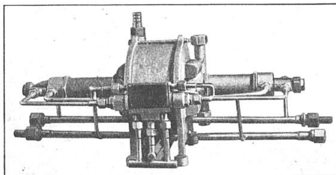
L'AUTO-PROPULSEUR « A. M. »
