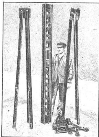
FIG. 2. — LE PONT DÉMONTÉ
