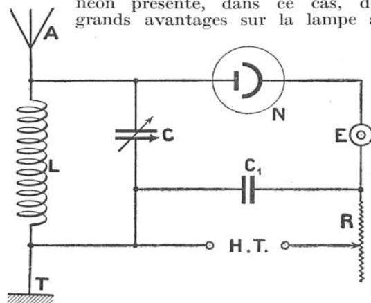
FIG. 4. — MONTAGE D'UNE LAMPE AU NÉON COMME DÉTECTRICE
