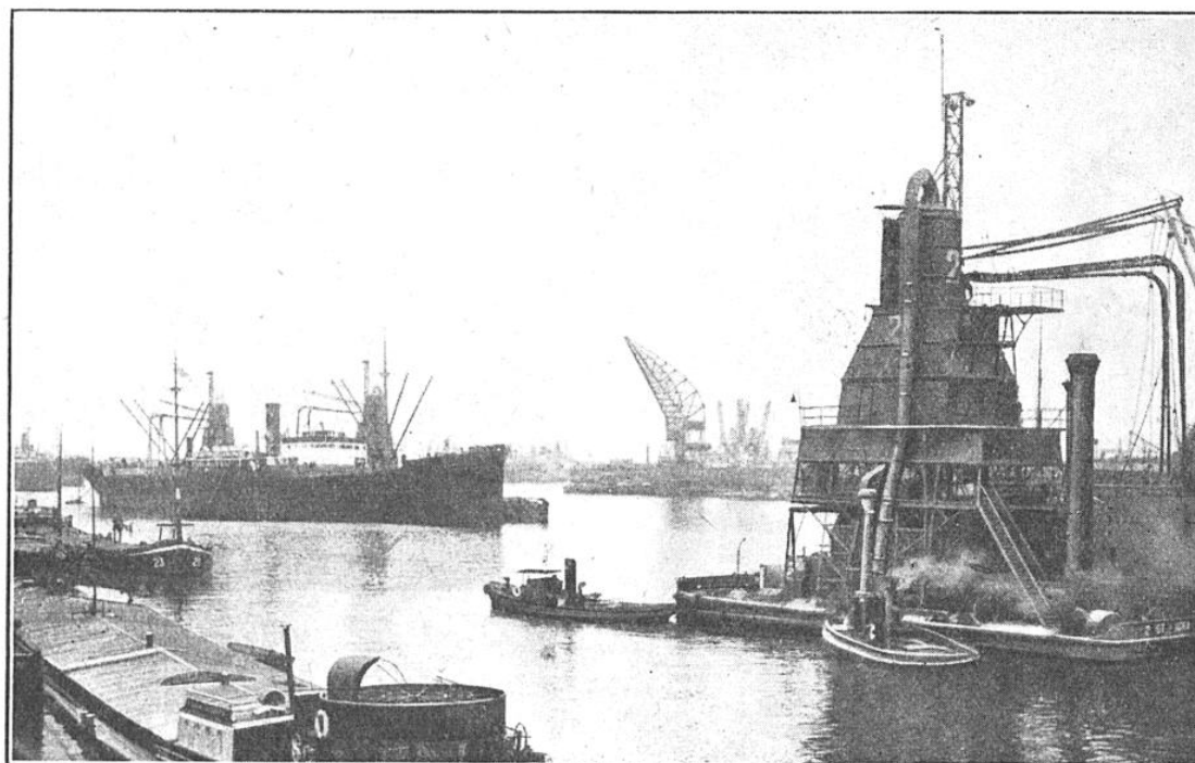
VUE DU BASSIN-CANAL DANS LE PORT D'ANVERS Au premier plan à droite, on aperçoit un très puissant élévateur pneumatique pour les grains.
