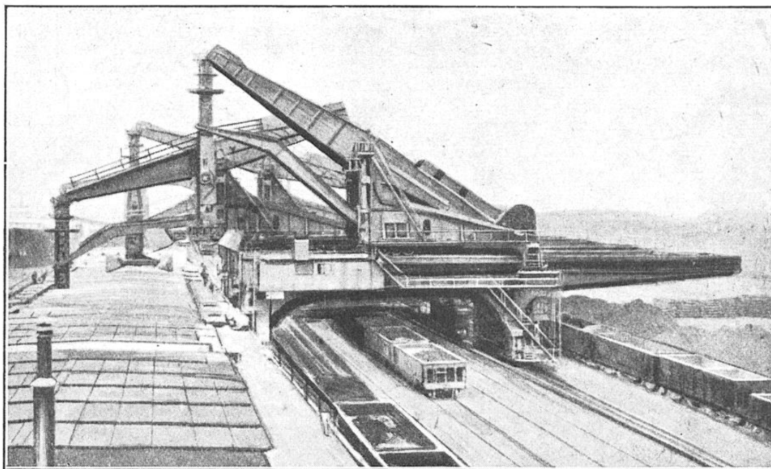
DÉCHARGEURS AUTOMATIQUES DE MINÉRAIS (SYSTÈME HULETT) ÉTABLIS PAR « THE WELLMANN SEAVAR MORGAN CO. », DE CLEVELAND (OHIO)
