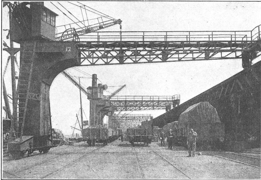
GRUES A DEMI-PORTIQUE DES NOUVEAUX QUAIS DU SUD A ANVERS
