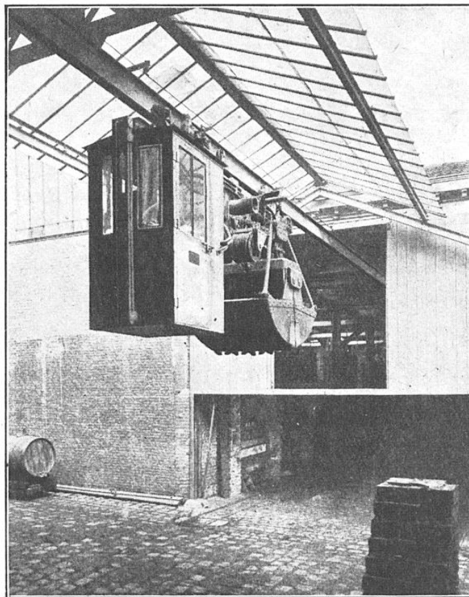
GUIDÉE PAR L'EMPLOYÉ SITUÉ DANS LA CABINE, LA BENNE TRANSPORTE RAPIDEMENT SA CHARGE
