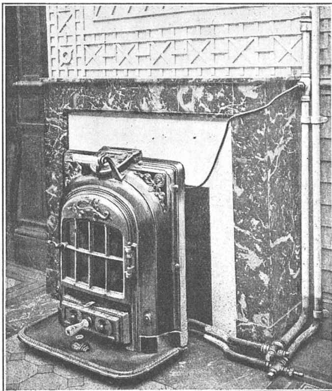
UNE SALAMANDRE INSTALLÉE POUR RÉALISER LE CHAUFFAGE CENTRAL D'UN APPARTEMENT OU D'UNE VILLA
