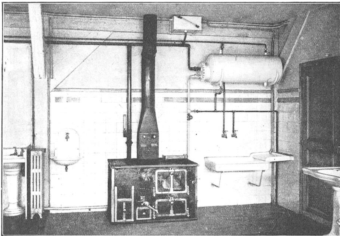
LE CHAUFFAGE CENTRAL PAR LE FOURNEAU DE CUISINE D. R. C.
