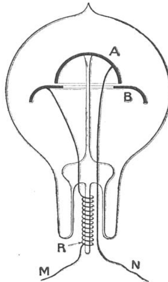
FIG. 1. — COUPE D'UNE LAMPE AU NÉON DITE « VEILLEUSE »
