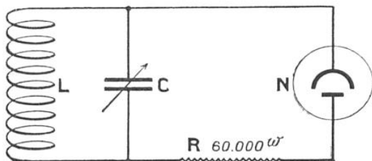
FIG. 3. — UN ONDEMÈTRE AU NÉON
