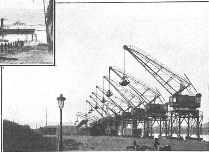
LES DIX GRUES DE 2,5 TONNES FOURNIES A LA CHAMBRE DE COMMERCE DE ROUEN
