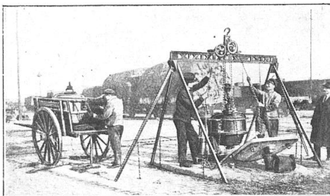
FIG. 1. — LE PONT UTILISÉ POUR LA MISE EN PLACE D'UN MOTEUR DE CABESTAN DANS UNE GARE
