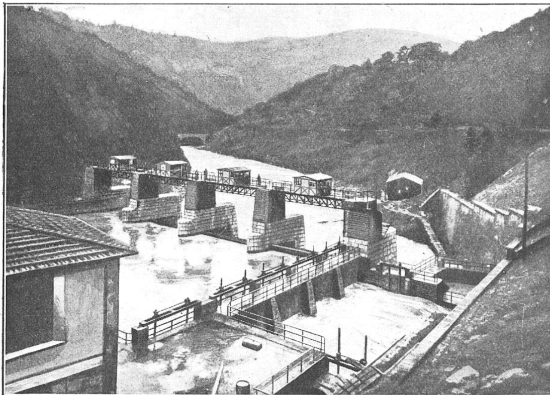
BARRAGE ET PRISE D'EAU DE LA CENTRALE HYDROÉLECTRIQUE DU SERCHIO (HTE-ITALIE)
