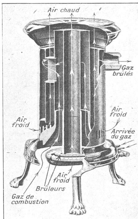
RADIATEUR A GAZ « LE CALORIC »
