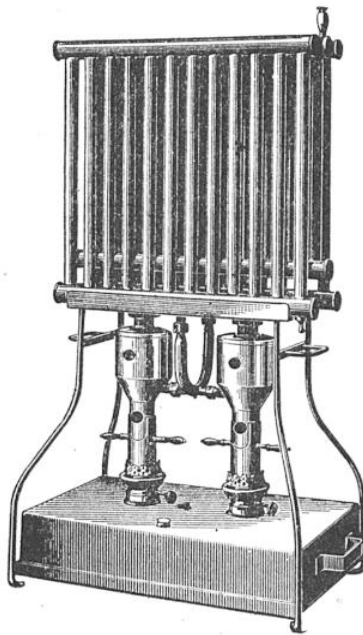
LE « SORCIER » Ce radiateur est chauffé par une lampe à pétrole ordinaire. Notre dessin ci-contre en montre la construction. Il se fait à un, deux ou trois brûleurs et les radiateurs sont à double ou triple rangée de tubes en cuivre de dix, douze ou dix-huit tubes chaque.
