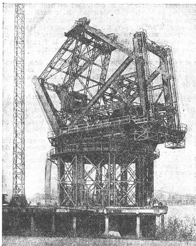
Montage de la grue de 250 tonnes fournie aux Chantiers de la Gironde (Bordeaux).
