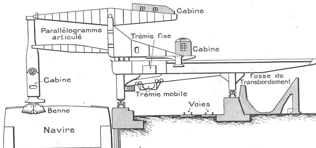
CROQUIS SCHÉMATIQUE D'UN APPAREIL HULETT, DE « THE WELLMANN SEAVAR MORGAN CO. »
