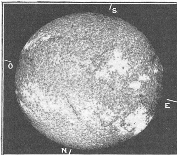
FIG. 8. — LE SOLEIL QUE NOS YEUX NE VOIENT PAS Photographie obtenue le 20 janvier 1926, par M. D'Azambuja, à l'aide du spectrohéliographe de l'Observatoire de Meudon, et montrant la couche supérieure des vapeurs de calcium dans l'atmosphère solaire.
