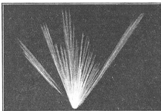
FIG. 4. — PHOTOGRAPHIE DE LA GRANDE COMÈTE DE 1861, DONT LA QUEUE EN ÉVENTAIL CONTIENT PLUSIEURS BRANCHES La tête des comètes, formée de fragments assez gros, subit l'attraction du Soleil, tandis que la queue, constituée par des corpuscules très petits, est repoussée par la lumière du Soleil.
