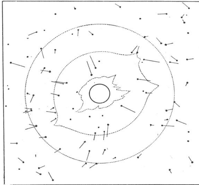
FIG. 9. — RÉGION DU CIEL PHOTOGRAPHIÉE PENDANT L'ÉCLIPSE DE SOLEIL DU 21 SEPTEMBRE 1922
