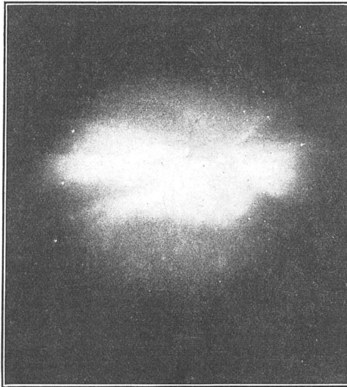
FIG. 5. — COURONNE D'AUORE BORÉALE PHOTOGRAPHIÉE LE 26 JANVIER 1926, A 19 H. 52 M., PAR M. LE PROFESSEUR CARL STÖRMER, A BYGDO, EN NORVÈGE A droite, les étoiles de la Constellation de Persée. A gauche, celles de la Constellation du Cocher.
