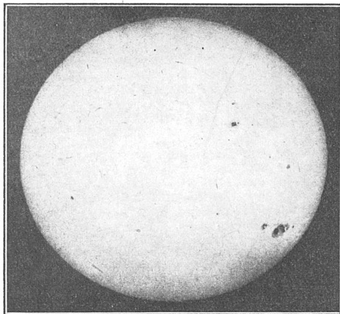
FIG. 7. — LE SOLEIL QUE NOS YEUX VOIENT Photographie directe, obtenue le 20 janvier 1926, à 14 h. 5 m., par M. Quénnisset, à l'Observatoire Flammarion de Juvisy.
