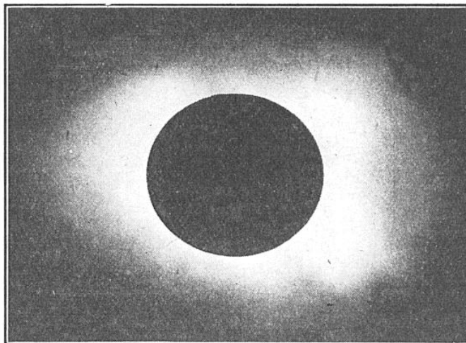
FIG. 3. — PHOTOGRAPHIE DE L'ÉCLIPSE TOTALE DE SOLEIL DU 8 JUIN 1918, MONTRANT AUTOUR DU DISQUE CENTRAL, ÉCLIPSÉ PAR LA LUNE, LA COURONNE SOLAIRE QUI N'EST OBSERVABLE QUE PENDANT LES ÉCLIPSES TOTALES. On peut concevoir l'existence de la couronne solaire comme le résultat de la répulsion exercée par la lumière du Soleil sur des particules extrêmement ténues, répulsion qui contre-balance exactement l'attraction de l'astre sur ces particules.
