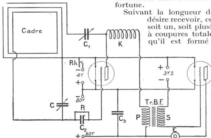
FIG. 6. — SCHÉMA D'UN RÉCEPTEUR PORTATIF
