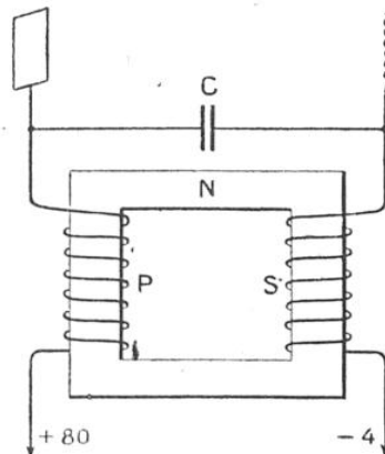
FIG. 8. — LE COUPLEUR BASSE FRÉQUENCE DONLE
