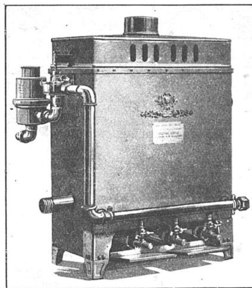
CHAUDIÈRE INTENSIVE « A. M. »
