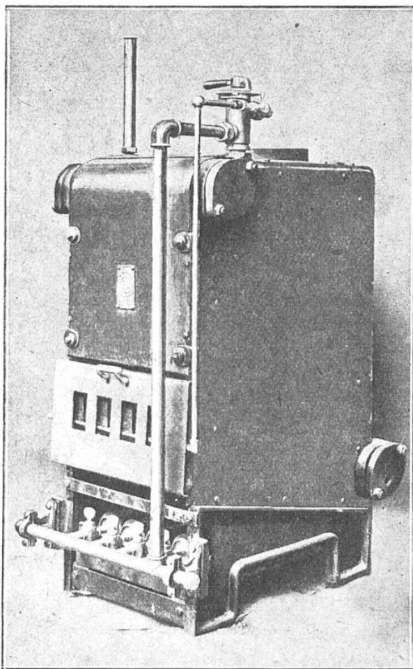
LA CHAUDIÈRE « PHI » A GAZ RÉSOUT TOUS LES PROBLÈMES DE CHAUFFAGE CENTRAL ET DE DISTRIBUTION D'EAU CHAUDE POUR APPARTEMENTS, VILLAS, MAGASINS, ATELIERS, ETC.
