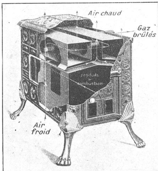
CALORIFÈRE A BOIS « LE CALORIC »
