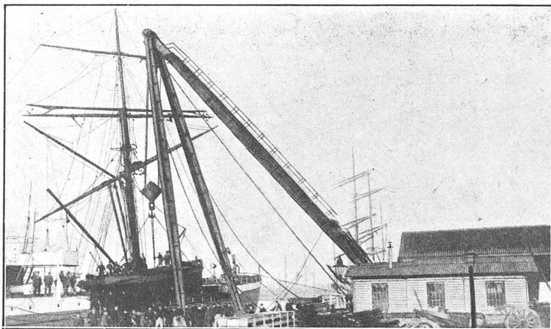
GRANDE BIGUE D'UNE PUISSANCE DE LEVAGE DE 120 TONNES, SUR LES QUAIS D'ANVERS Cette bigue s'élève à 29 mètres au-dessus du quai et peut déplacer, avec une oscillation de 13 mètres, des charges de 120 tonnes. Elle est pourvue d'un appareillage électrique.
