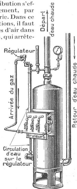
CHAUDIÈRE « C.R.T. » POUR LE CHAUFFAGE CENTRAL AU GAZ
