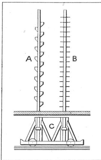
ANCIENS MATS UTILISÉS SUR LES GRANDES SCÈNES
