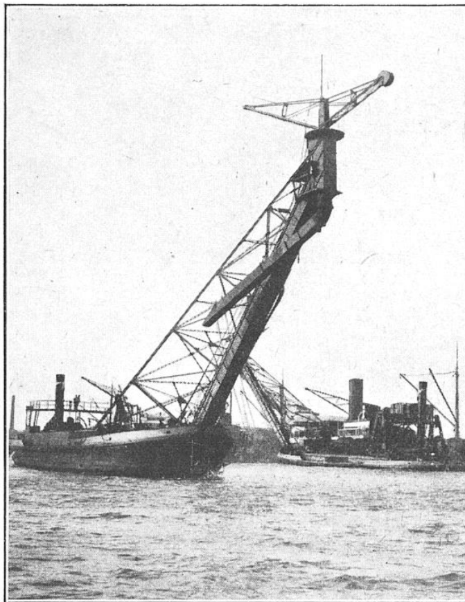
TRANSPORTEUR DE CHARBON AU PORT DE ROTTERDAM
