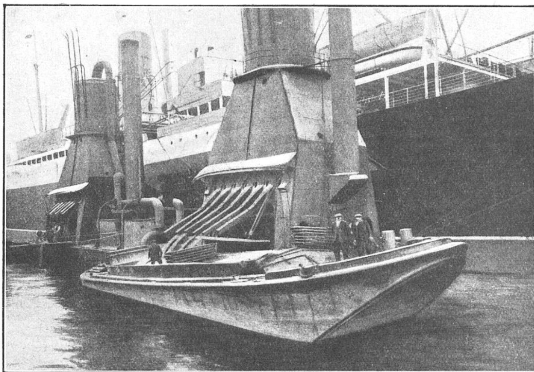
DÉCHARGEMENT DU BLÉ PAR ÉLÉVATEURS PNEUMATIQUES DANS LE PORT DE LONDRES
