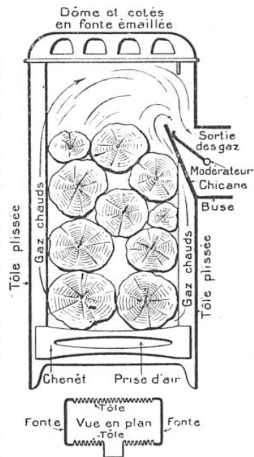
COUPE DU POËLE A BOIS « LE PIERROT »
