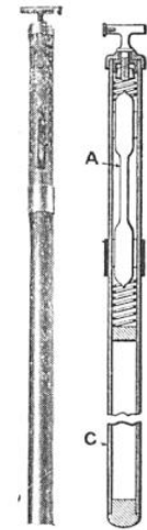
FIG. 3 LA PERCHE AU NÉON
