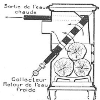
COUPE DU POËLE A BOIS « LE STYX » UTILISÉ POUR LE CHAUFFAGE CENTRAL
