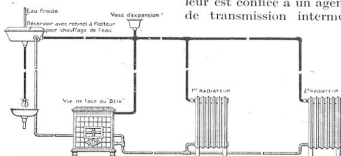
UNE INSTALLATION DE CHAUFFAGE CENTRAL RÉALISÉE DANS UN PETIT APPARTEMENT PAR LE POËLE A BOIS « STYX »
