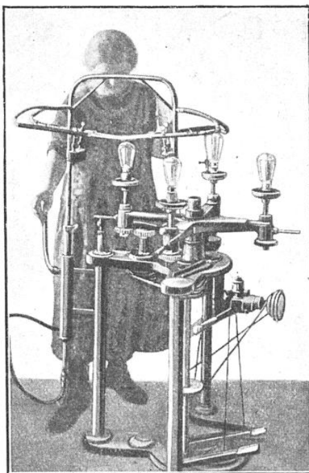
SUR CETTE MACHINE, QUATRE CHALUMEAUX RAMOLLISSENT LA POINTE DE LA LAMPE DE MANIÈRE À MÉNAGER UNE OUVERTURE, PAR LAQUELLE SE FERONT TOUTES LES MANIPULATIONS
