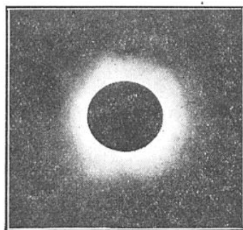
FIG. 8. — PHOTOGRAPHIE DE L'ÉCLIPSE DE SOLEIL DU 21 SEPTEMBRE 1922, PRISE A SANTHORPE (QUEENSLAND), PAR M. DAVID ROSS
