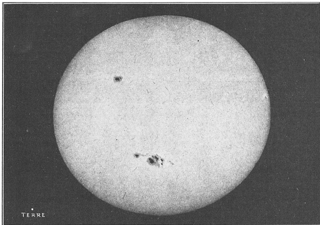
FIG. 2. — DIMENSIONS COMPARÉES DE LA TERRE ET DU SOLEIL
