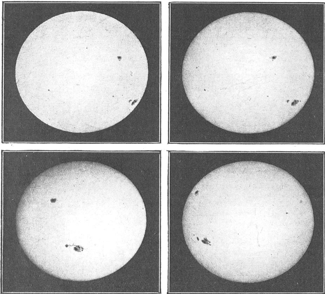
FIG. 3. — LA ROTATION DU SOLEIL RENDUE ÉVIDENTE PAR LE DÉPLACEMENT DES TACHES SUR SON DISQUE, PENDANT LEUR PASSAGE EN VUE DE LA TERRE
