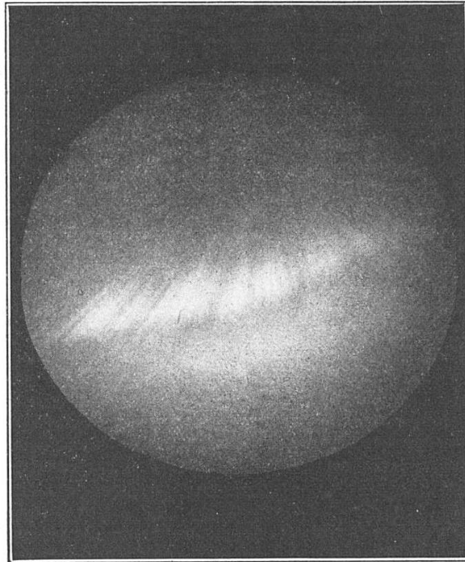
FIG. 6. — DRAPERIE D'AUORE BORÉALE VUE PRÈS DU ZÉNITH, A BYGDO, LE 27 JANVIER 1926, A 2 HEURES DU MATIN
