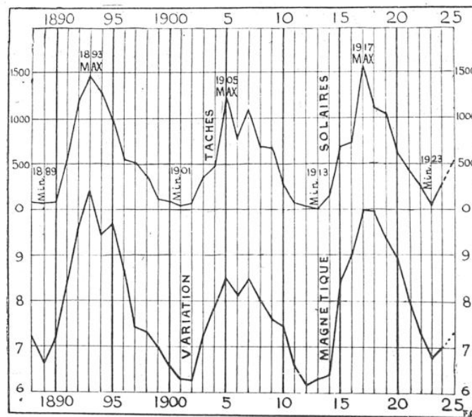
FIG. 4. — COURBES MONTRANT LA CONCORDANCE ENTRE L'ACTIVITÉ SOLAIRE ET LE MAGNÉTISME TERRESTRE DEPUIS TRENTE-CINQ ANS
