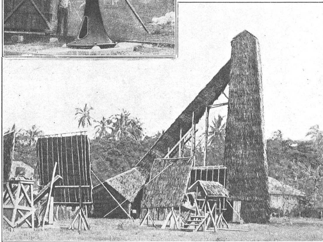
FIG. 7. — UNE EXPÉDITION SCIENTIFIQUE S'EST RENDUE AUX ILES DE LA SONDE POUR OBSERVER UNE RÉCENTE ÉCLIPSE DE SOLEIL.
