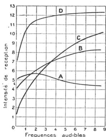
FIG. 9. — COURBES D'ÉTUDES DE DIVERS SYSTÈMES DE COUPLAGE ENTRE ÉTAGES BASSE FRÉQUENCE
