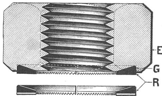
COUPE DE NOUVEL ÉCROU
