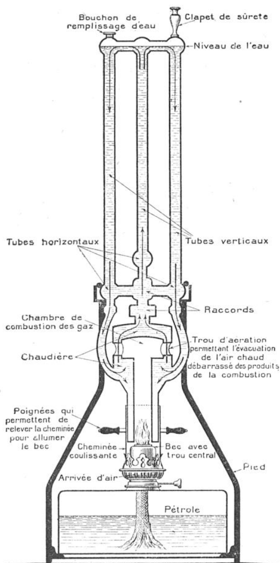
RADIATEUR A PÉTROLE OU A ESSENCE LE « SORCIER »
