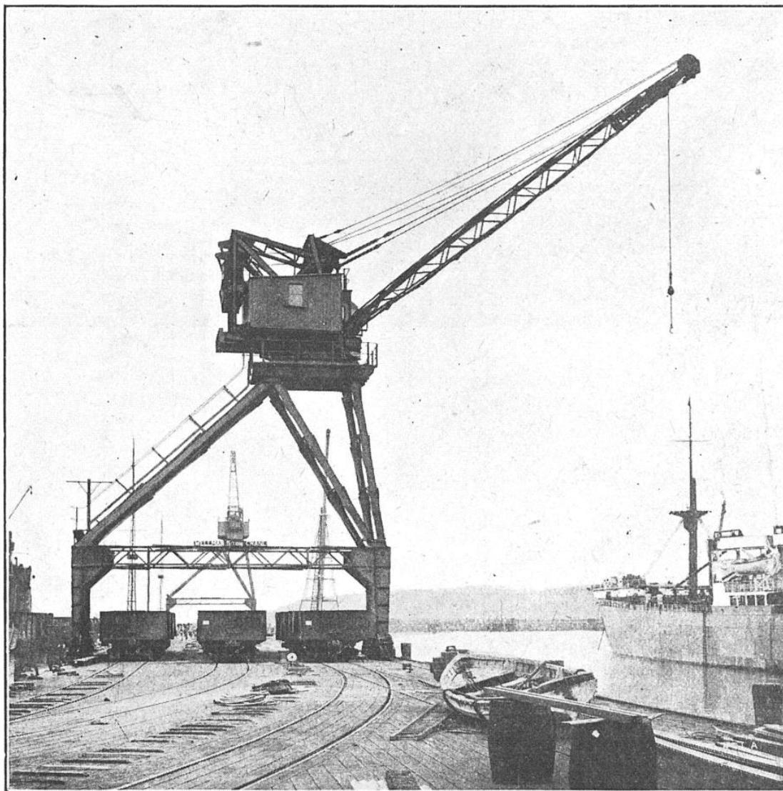
UNE GRUE DE 50 TONNES DU PORT DE LONDRES
