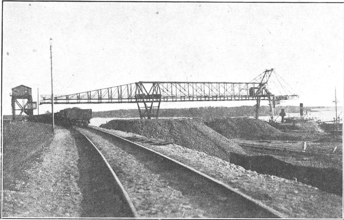
GRANDE GRUE PORTIQUE DE « THE BROWN HOISTING MACHINERY CO. », DE CLEVELAND (OHIO), A OXELOSUND (SUÈDE)
