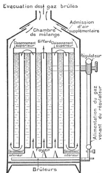
SCHÉMA DU FONCTIONNEMENT DE LA CHAUDIÈRE INTENSIVE « A. M. »
