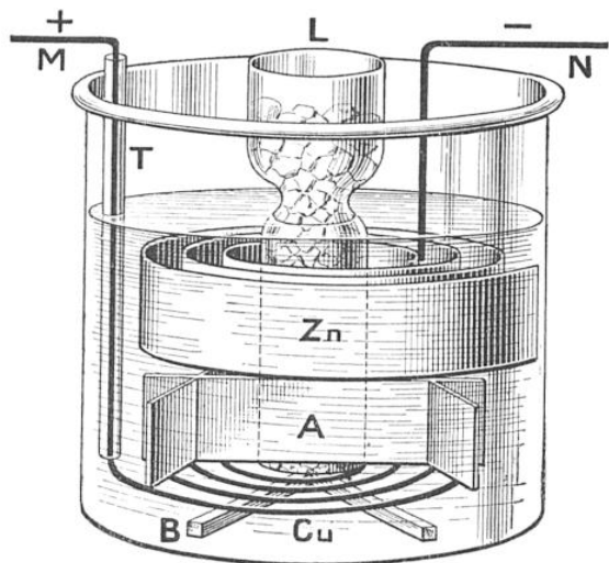
FIG. 7. — ÉLÉMENT DE PILE AU SULFATE DE CUIVRE
