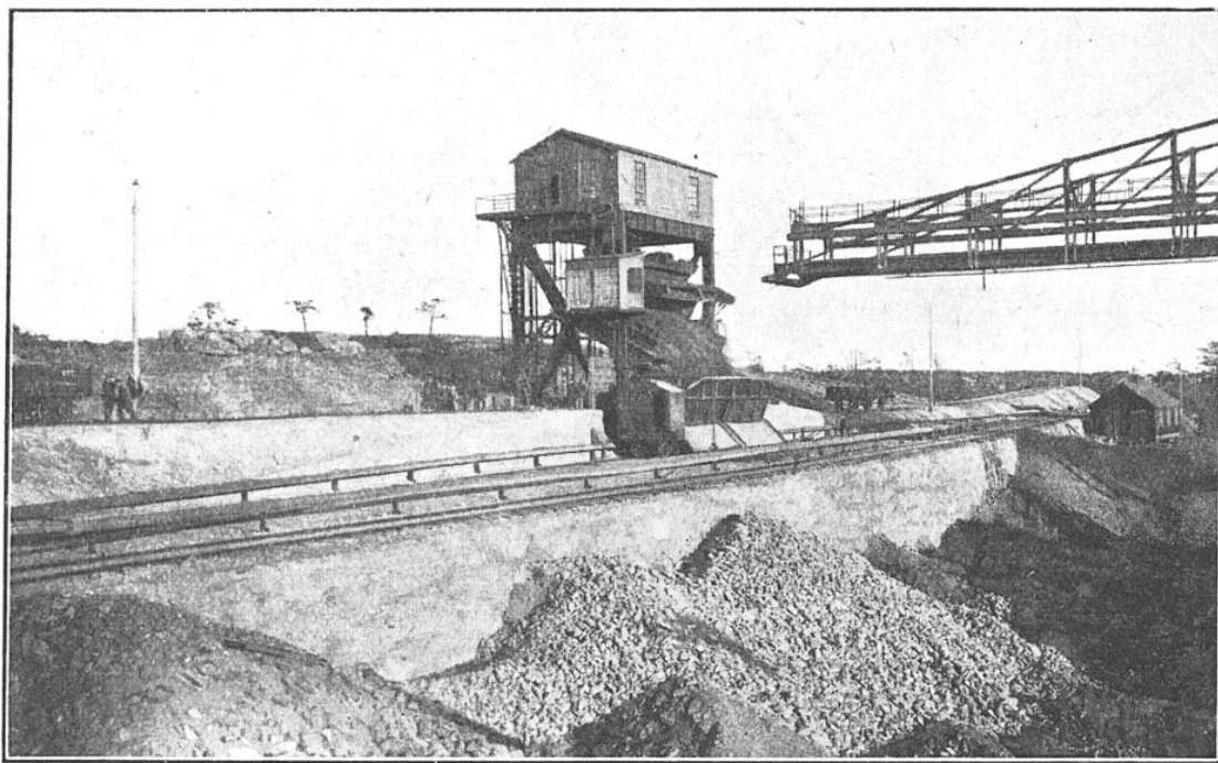
BASCULEUR A OXELOSUND (SUÈDE), POUR LE DÉCHARGEMENT DE WAGONS DE 30 TONNES Ces wagons sont vidés par un culbuteur dans un wagon de manutention de 60 tonnes et le minerai ensuite déversé le long du mur du parc de stockage. Il est ensuite repris par la grue portique et transféré au dépôt quand aucun bateau n'est à charger immédiatement.
