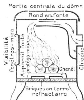
COUPE DU POËLE A BOIS « FAUNUS »
