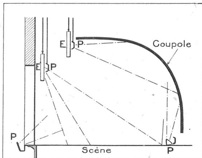
SCHEMA DE LA COUPOLE DIFFUSANTE FORTUNY
