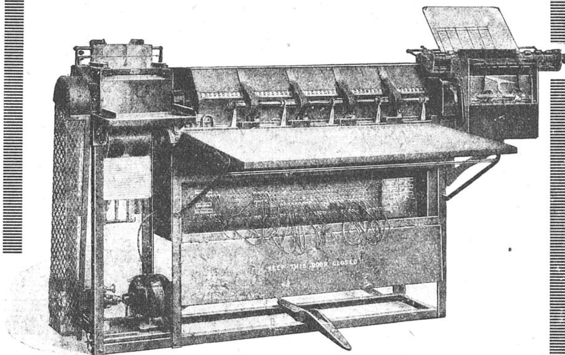
UN DES ÉLÉMENTS "HOLLERITH" : LA TABULATRICE IMPRIMANTE
