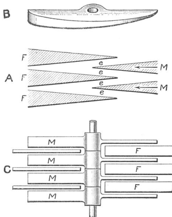
FIG. 4. — SCHÉMA DU CONDENSATEUR
