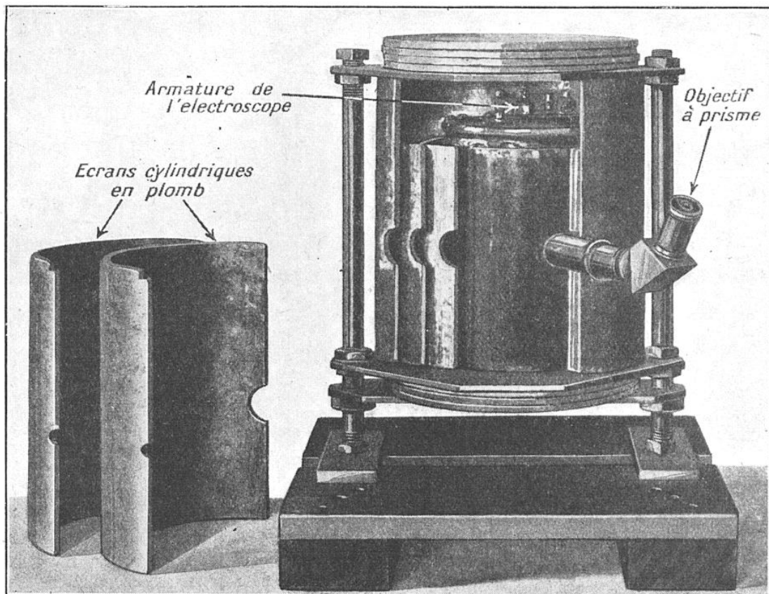
DÉTAILS DE L'ÉLECTROSCOPE DE MILLIKAN AVEC LES ÉCRANS CYLINDRIQUES FORMÉS PAR DES FEUILLES DE PLOMB. LES DÉVIATIONS SONT OBSERVÉES AU MOYEN DE LA LUNETTE A PRISME DE DROITE
