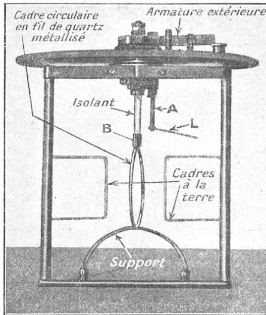
LE MÉCANISME INTÉRIEUR DE L'ÉLECTROSCOPE UTILISÉ PAR MILLIKAN
