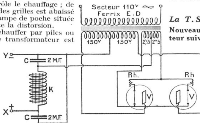
FIG. 3. — TABLEAU D'ALIMENTATION DE TENSION-PLAQUE PAR LE COURANT ALTERNATIF
