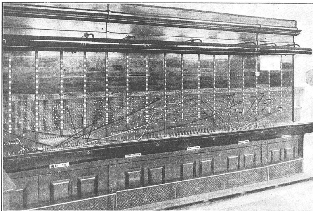
UN MEUBLE DE TÉLÉPHONE MANUEL ORDINAIRE MONTRANT LES INEXTRICABLES COMBINAISONS DE LIGNES QUE DOIVENT RÉALISER LES OPÉRATRICES AU HASARD DES APPELS
