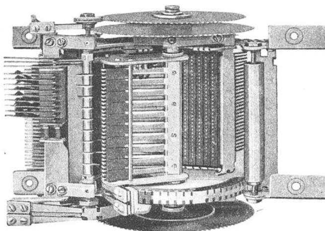
TYPE DU SÉLECTEUR FINAL AYANT POUR FONCTION LA RECHERCHE DE LA LIGNE PROPRE DE L'ABONNÉ APPELÉ
