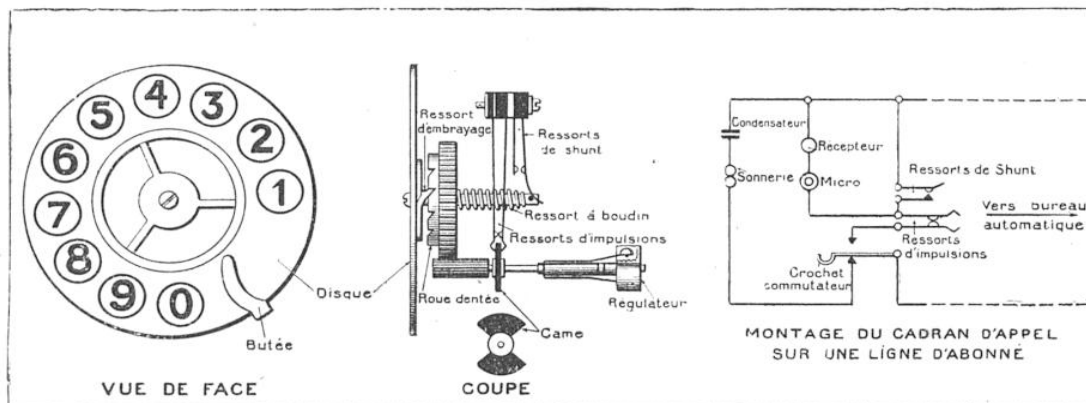
SCHEMA DU MECANISME D'APPEL AUTOMATIQUE
