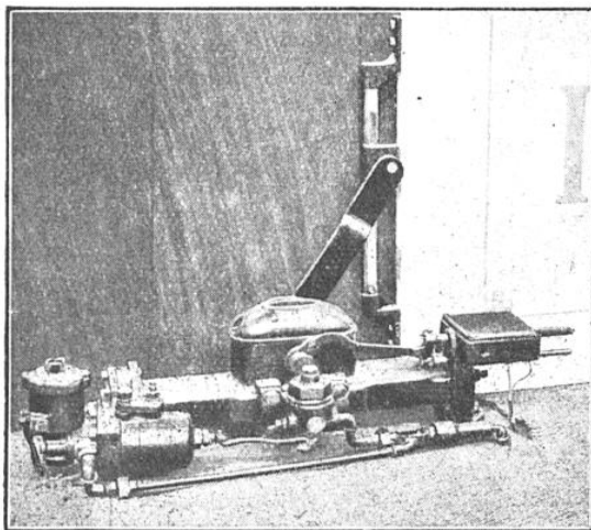
DÉTAIL DU MÉCANISME DE COMMANDE
