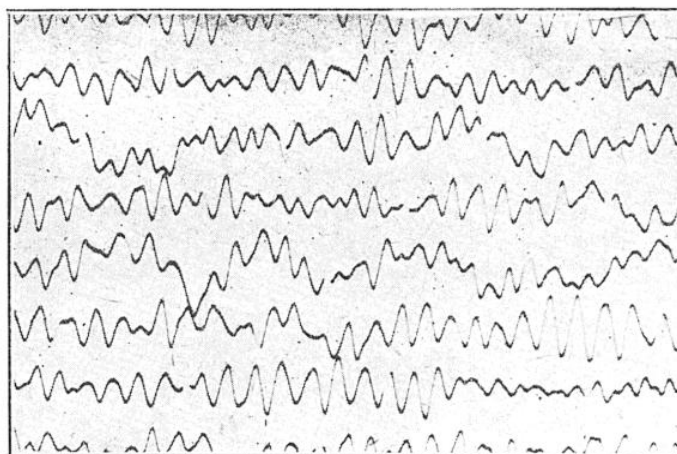
FIG. 3. - MOUVEMENTS MICRO-SÉISMQUES DANS LESQUELS APPARAÎT UNE ONDULATION ASSEZ LENTE (PÉRIODE 30 SECONDES) DUE À L'ACTION DU VENT, EN MÊME TEMPS QU'UN MOUVEMENT PLUS RAPIDE ASSEZ MARQUÉ (COMPOSANTE VERTICALE)
