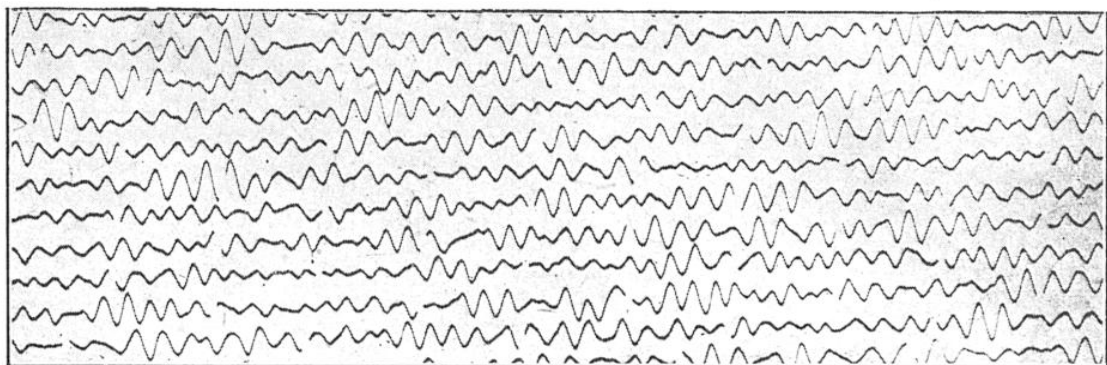
FIG. 1. — DANS SES FRÉMISSEMENTS, LE SOL A DES MOUVEMENTS VERTICAUX DONT LES OSCILLATIONS DÛRENT ENVIRON SEPT SECONDES ET DONT L'AMPLITUDE NE DÉPASSE PAS QUELQUES MILLIÈMES DE MILLIMÈTRE
