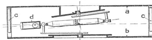
DISPOSITIF EMPLOYÉ POUR REPRÉSENTER LES MOUVEMENTS DE MERCURE
