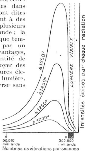
FIG. 11. — ÉMISSION DES CORPS SOLIDES A DIVERSES TEMPÉRATURES
