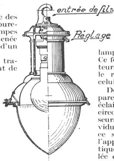
DEMI-COUPÉ D'UN APPAREIL POUR L'ÉCLAIRAGE INTÉGRAL
