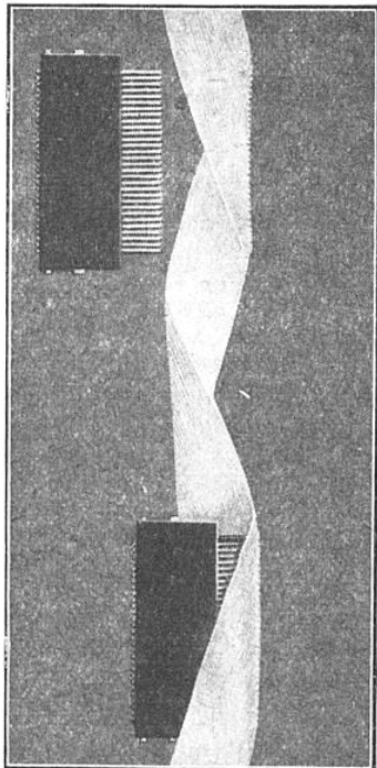
UN RUBAN TÉLÉPHONIQUE Ce ruban contient trente fils téléphoniques qui sont dénudés sur l'arête des plis représentés. Une réglette en forme de peigne vient cueillir chaque fil sur l'une de ses dents. Par l'autre face, cette réglette se fixe sur le sélecteur.
