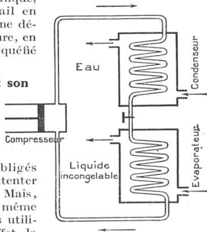
FIG. 13. — PRINCIPE DE LA MACHINE FRIGORIFIQUE A GAZ LIQUÉFIÉ L'ammoniaque (par exemple) est comprimée, puis envoyée (flèche supérieure) dans le serpentin du « condenseur », où elle se liquéfie ; elle s'évapore ensuite dans l'« évaporateur » en refroidissant le « liquide incongélable », puis elle retourne au compresseur (flèche inférieure).
