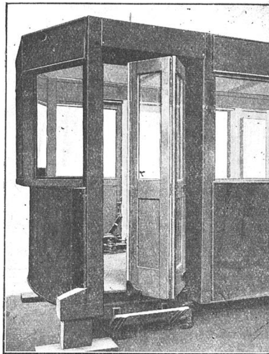
COMMENT S'OUVRE LA PORTE DU TRAMWAY FAITE DE DEUX VANTAUX ASSEMBLÉS
