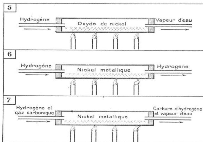
LE PROCÉDÉ D'HYDROGÉNATION CATALYTIQUE DES PROFESSEURS SABATIER ET SENDERENS
