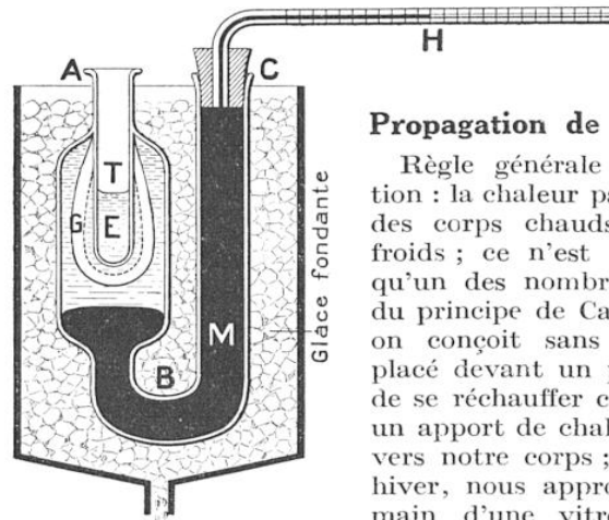
FIG. 10. — CALORIMÈTRE
