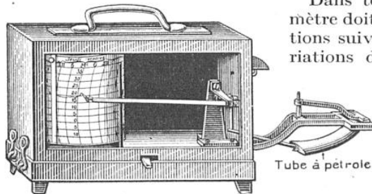
FIG. 5. — THERMOGRAPHE Grâce à cet appareil on peut enregistrer les températures de toute une semaine.
