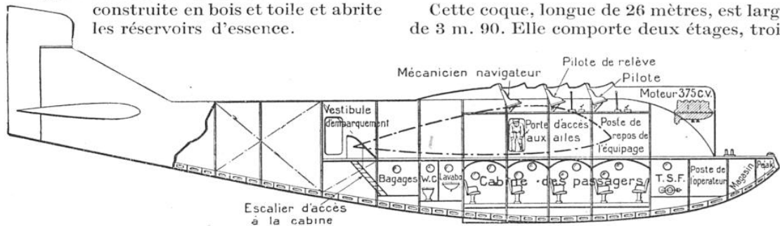
COUPE LONGITUDINALE DU NOUVEL HYDRAVION
