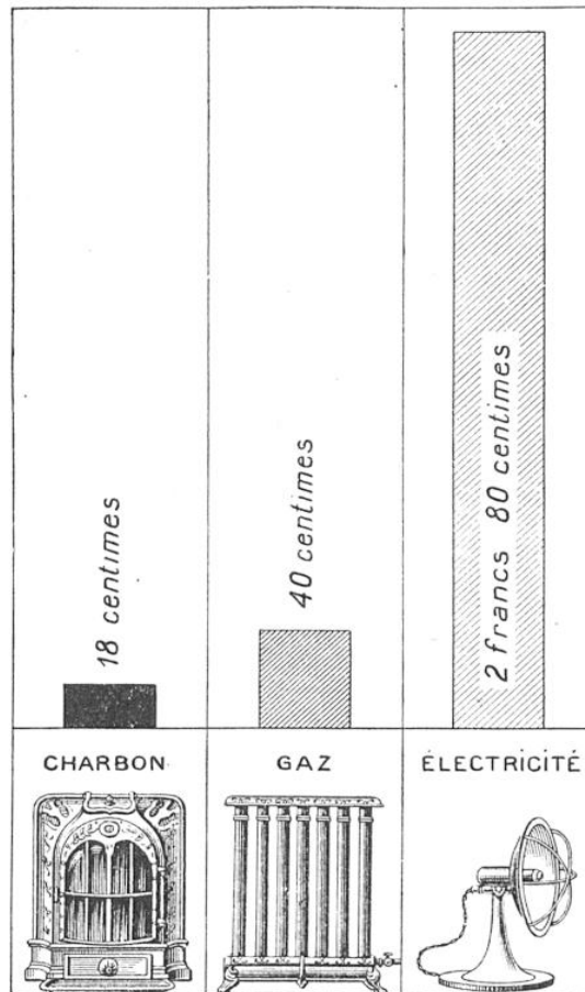
FIG. 12. — DÉPENSE HORAIRE POUR LE CHAUFFAGE D'UNE PETITE PIÈCE (30 M 3 ) Les prix de base (premier semestre 1926) sont : 550 francs la tonne de charbon, 0 fr. 75 le mètre cube de gaz et 12 centimes l'hectowatt-heure d'énergie électrique.
