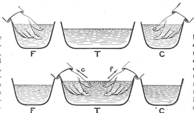
FIG. 1 ET 2. — RELATIVITÉ DES SENSATIONS THERMIQUES
