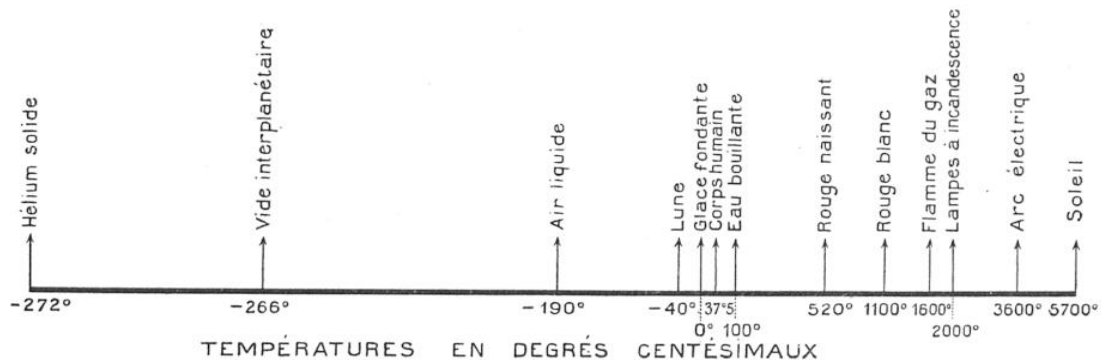
FIG. 9. — LES TEMPÉRATURES EXTRÊMES DU SYSTÈME SOLAIRE
