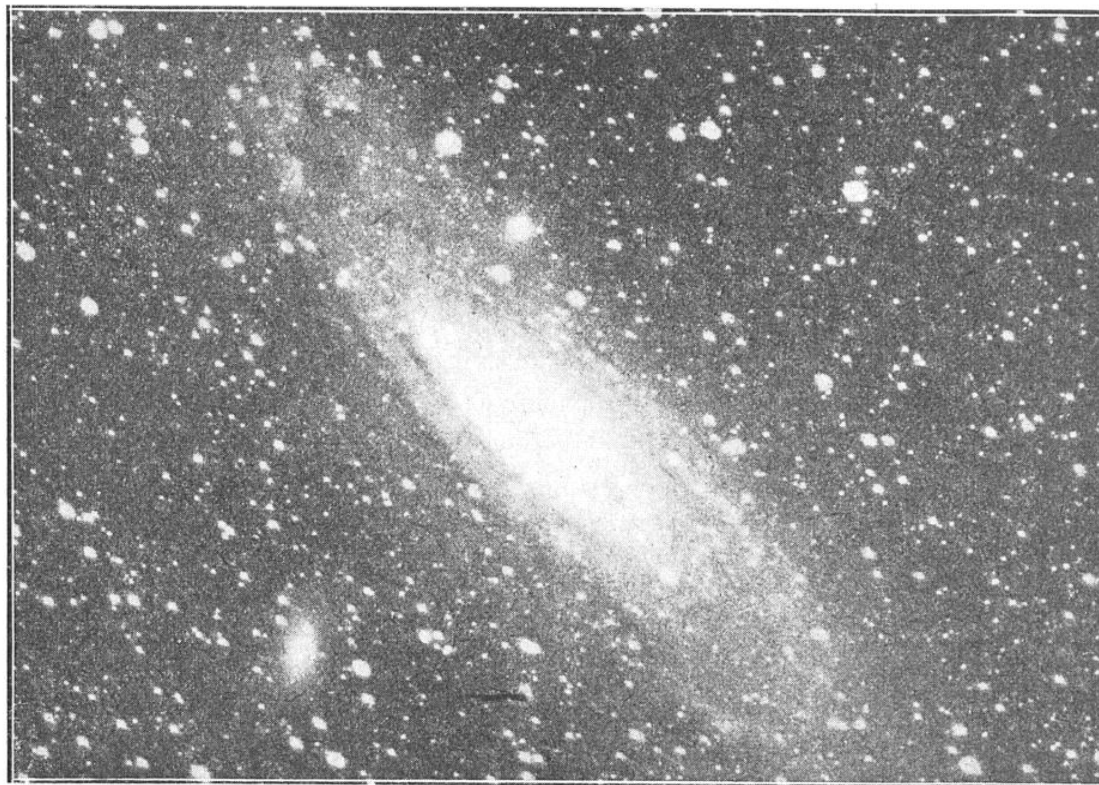
LA CÉLÈBRE NÉBULEUSE SPIRALE D'ANDROMÈDE
