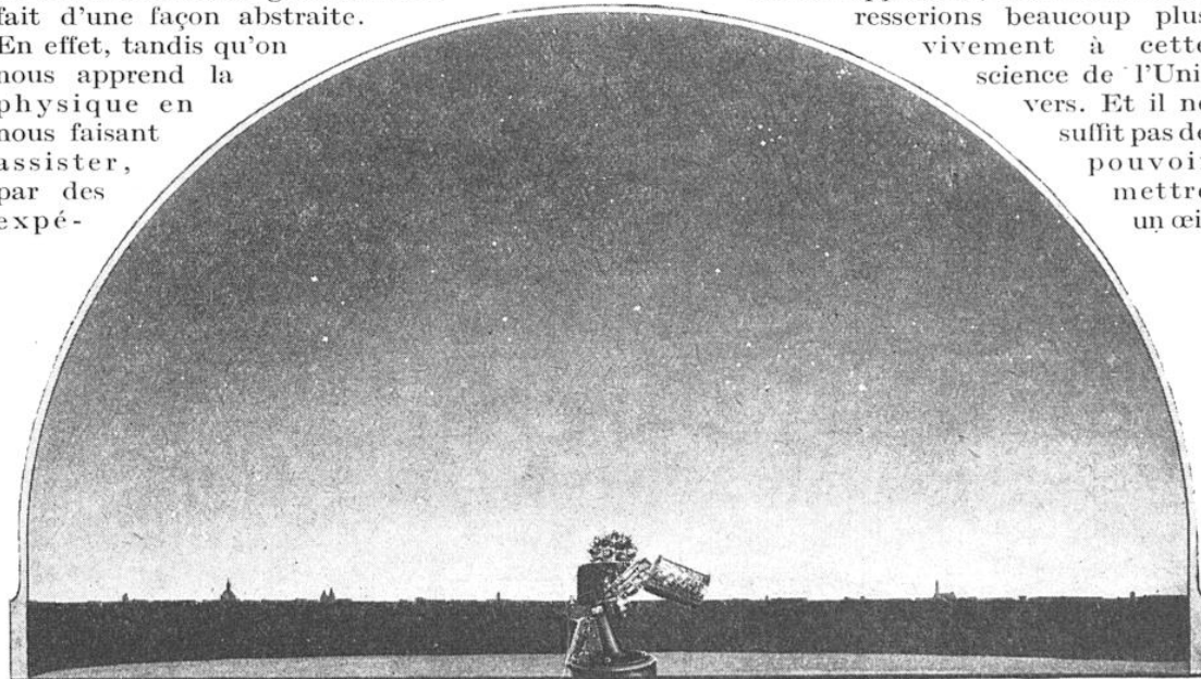
INSTALLÉ AU CENTRE D'UNE DEMI-SPHÈRE DE 10 MÈTRES DE DIAMÈTRE, L'APPAREIL CI-DESSUS PROJETTE À L'INTÉRIEUR DE CETTE COUPOLE TOUTES LES CONSTELLATIONS, LES PLANÈTES, LE SOLEIL, LA LUNE, AVEC LEURS MOUVEMENTS RESPECTIFS
