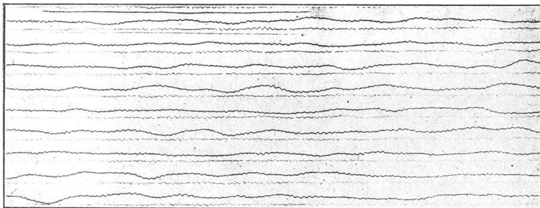
FIG. 4. — MOUVEMENTS MICROSÉISMQUES ANALOGUES AUX PRÉCÉDENTS, MAIS OÙ LE MOUVEMENT RAPIDE EST MOINS ACCENTUÉ (PÉRIODES 30 SECONDES ET 4,5 SECONDES. COMPOSANTE HORIZONTALE)
