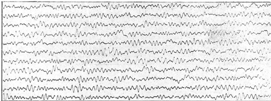
FIG. 5. — AGITATION MICROSÉISMIQUE DU TYPE LE PLUS FRÉQUENT (PÉRIODE D'ENVIRON SIX SECONDES)
