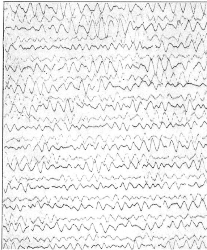
FIG. 2. — COURBES REPRÉSENTANT LES MOUVEMENTS HORIZONTAUX DU SOL (DEUX COMPOSANTES NORD-SUD ET EST-OUEST) DONT LES PÉRIODES ET LES AMPLITUDES SONT À PEU PRÈS LES MÊMES QUE CELLES DES MOUVEMENTS VERTICAUX (FIG. 1)
