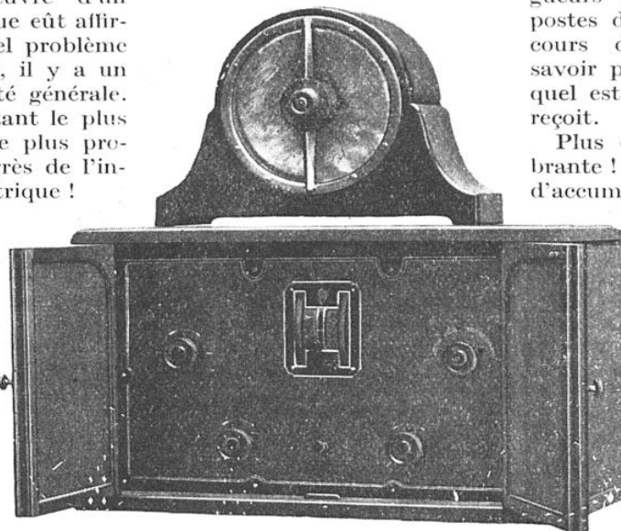
LE RÉCEPTEUR SFER 20 AVEC HAUT-PARLEUR « RADIO-LAVOX » FORME PENDULE
