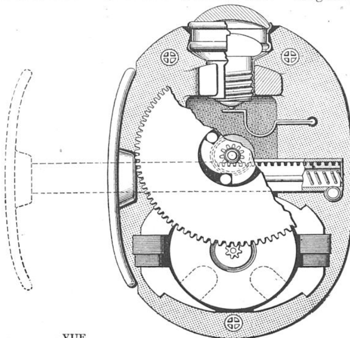
VUE EN COUPE DE LA LAMPE ÉLECTROMÉCANIQUE DE POCHE
