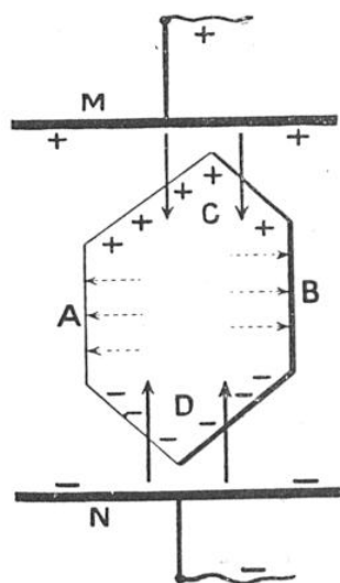
FIG. 1. — ACTION D'UN CHAMP ÉLECTRIQUE SUR UN CRISTAL DE QUARTZ TAILLÉ PERPENDICULAIREMENT À L'AXE OPTIQUE
