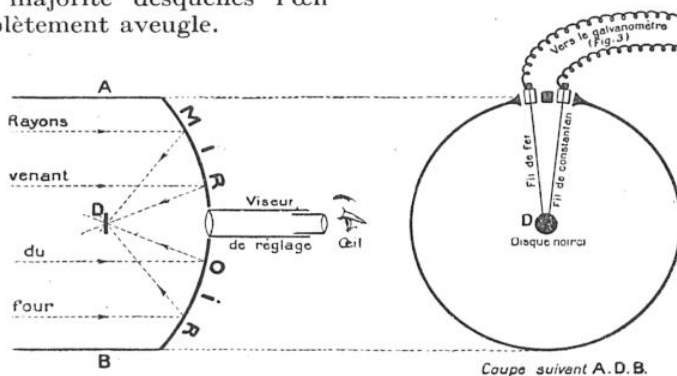
FIG. 4. — TÉLESCOPE PYROMÉTRIQUE
