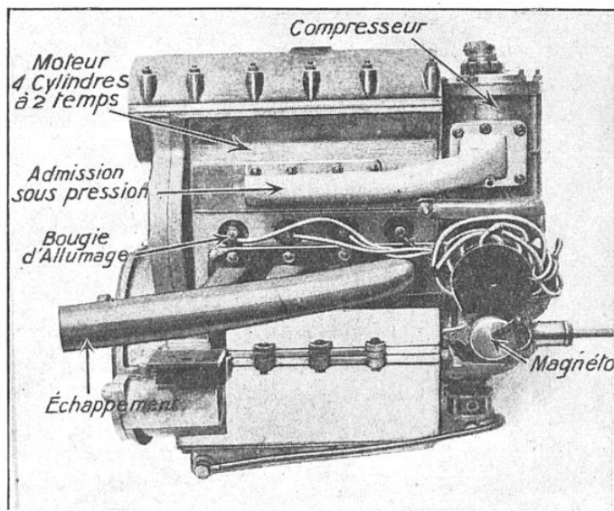
FIG. 6. — MOTEUR A DEUX TEMPS COZETTE, ALIMENTÉ PAR COMPRESSEUR ROTATIF
