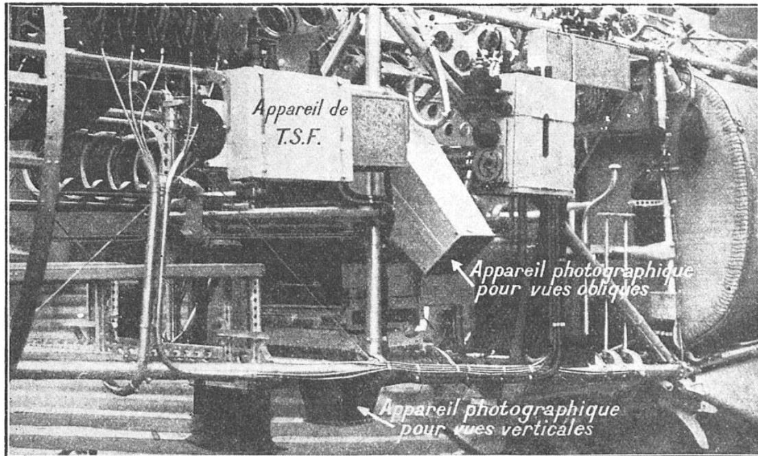
FIG. 8. — INSTALLATION D'APPAREILS PHOTOGRAPHIQUES, POUR VUES VERTICALES ET OBLIQUES, A BORD D'UN AVION
