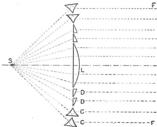
FIG. 1. — LE PERFECTIONNEMENT APPORTÉ AUX PHARES PAR FRESNEL
