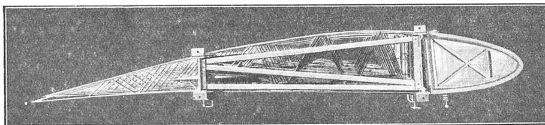
PROFIL D'UNE AILE MONTRANT L'EMPLACEMENT, A L'AVANT, DES NOURRICES D'ESSENCE
