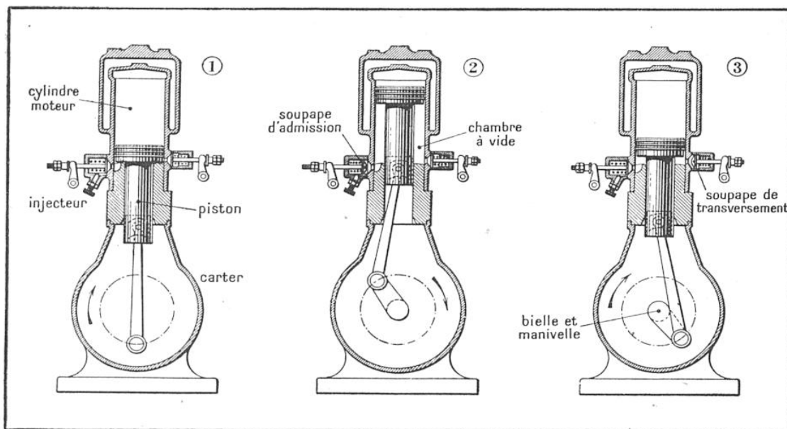
FIG. 4. — COUPES SCHÉMATIQUES MONTRANT LE FONCTIONNEMENT DU MOTEUR DE MONTAZET ET JOHANSON, PAR ATOMISATION DU PÉTROLE OU DU GASOIL
