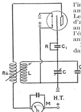
FIG. 5. — MONTAGE DU QUARTZ DANS UN OSCILLATEUR QU'IL CONTRÔLE, POUR ÉTUDE DE LA COURBE DE RÉSONANCE DU CRISTAL
