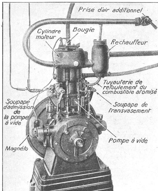
FIG. 5. — LE MOTEUR D'ÉTUDE DE MONTAZET ET JOHANSON POUR L'UTILISATION DES COMBUSTIBLES LOURDS : PÉTROLE ET HUILES MINÉRALES OU VÉGÉTALES
