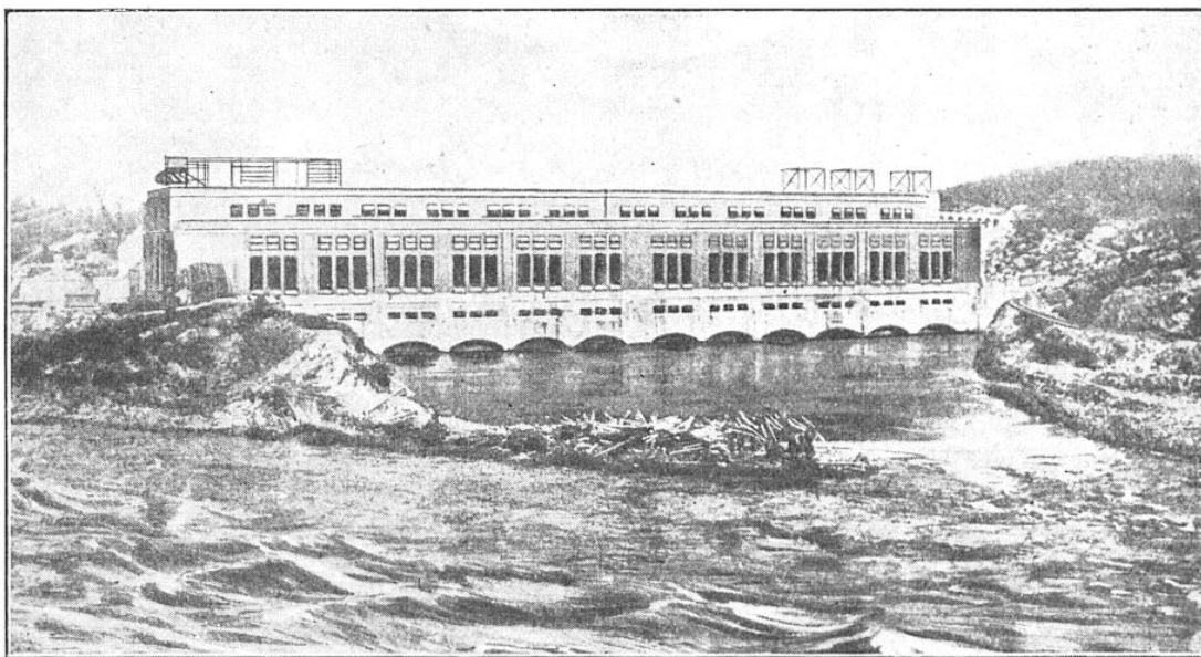
VUE AVANT DE LA CENTRALE HYDROÉLECTRIQUE DE L'ÎLE MALIGNE
