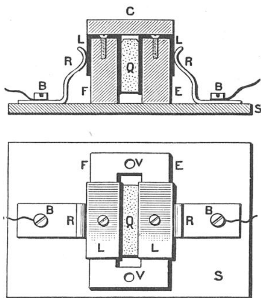
FIG. 3. — COUPE ET PLAN (COUVERCLE ENLEVÉ) DU MONTAGE DU CRISTAL
