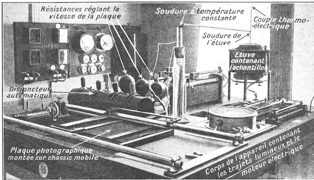
APPAREIL ENREGISTREUR MESURANT LA DILATATION DES VERRES
