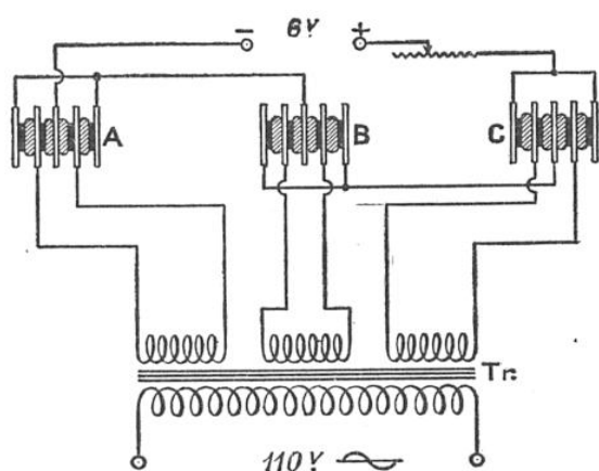
FIG. 8. — MONTAGE COMMERCIAL D'UN RECTIFICATEUR RUBEN
