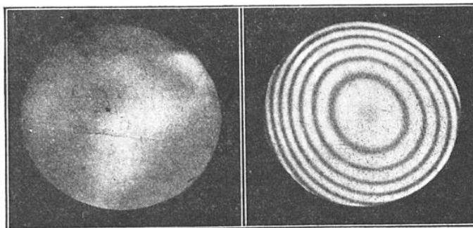
MÉTHODE DE VÉRIFICATION DES MIROIRS D'OPTIQUE
