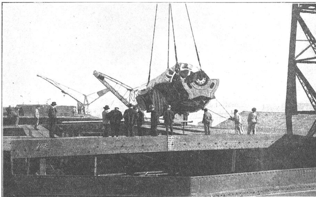
LA TURBINE ARRIVE SUR LE PONT DE L'« ILE-DE-FRANCE »
