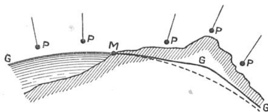
FIG. 2. — LA SURFACE DU GÉOÏDE « G » EST, EN CHAQUE POINT, PERPENDICULAIRE A LA DIRECTION DU FIL À PLOMB « P »
