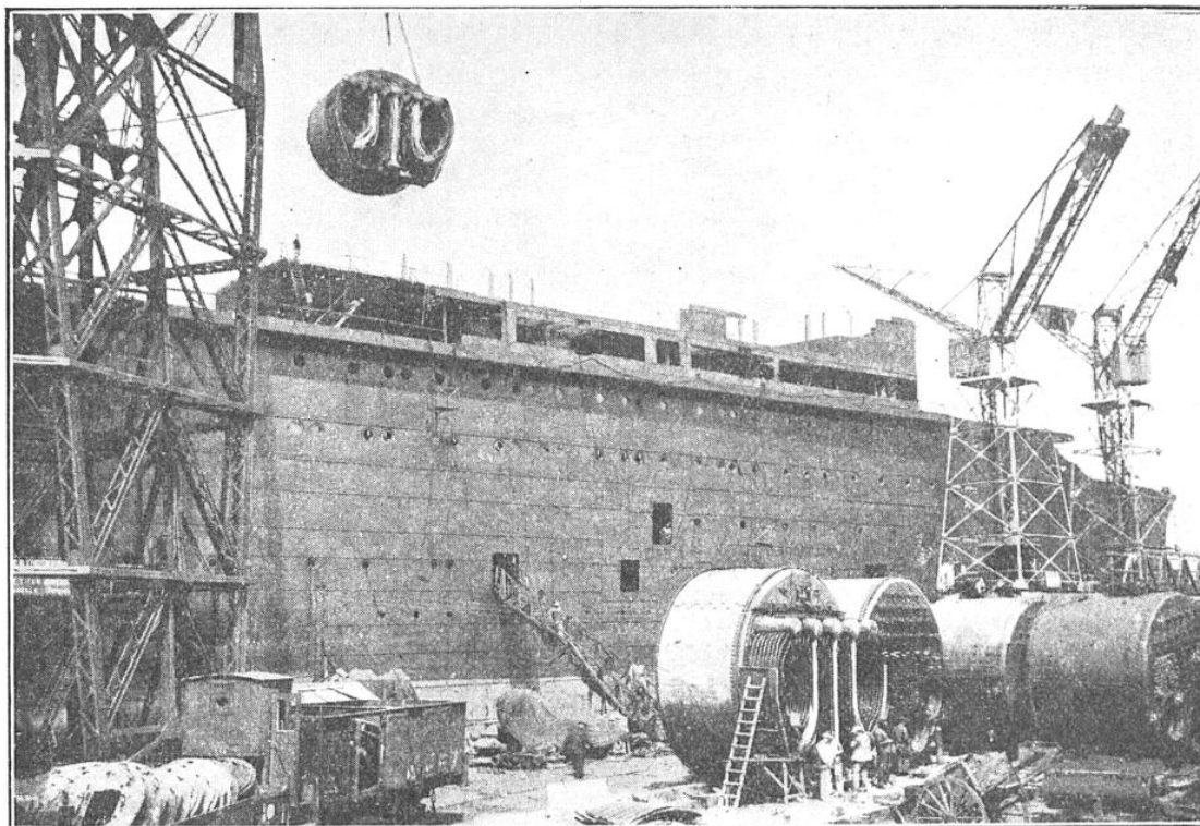
EMBARQUEMENT D'UN ÉLÉMENT DE CHAUDIÈRE
