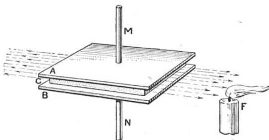
FIG. 4. — ACTION MÉCANIQUE DU QUARTZ OSCILLANT DANS UN CHAMP ALTERNATIF INTENSE
