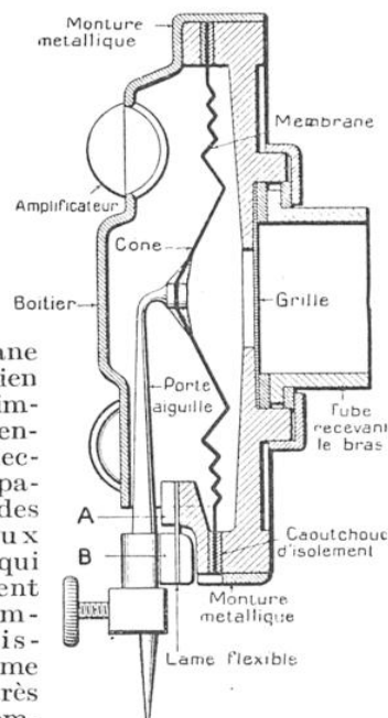
COUPE DE L'APPAREIL « MIRAPHONIC »
