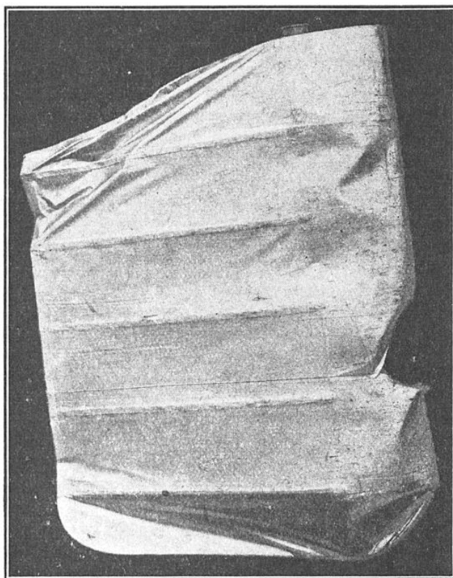
VUE DE PROFIL ET DE FACE DU GOUVERNAIL DE DIRECTION, QUE LE TRAIN DE DÉMARRAGE, LACHÉ TROP TOT, EST VENU SECTIONNER, CAUSANT AINSI L'ACCIDENT
