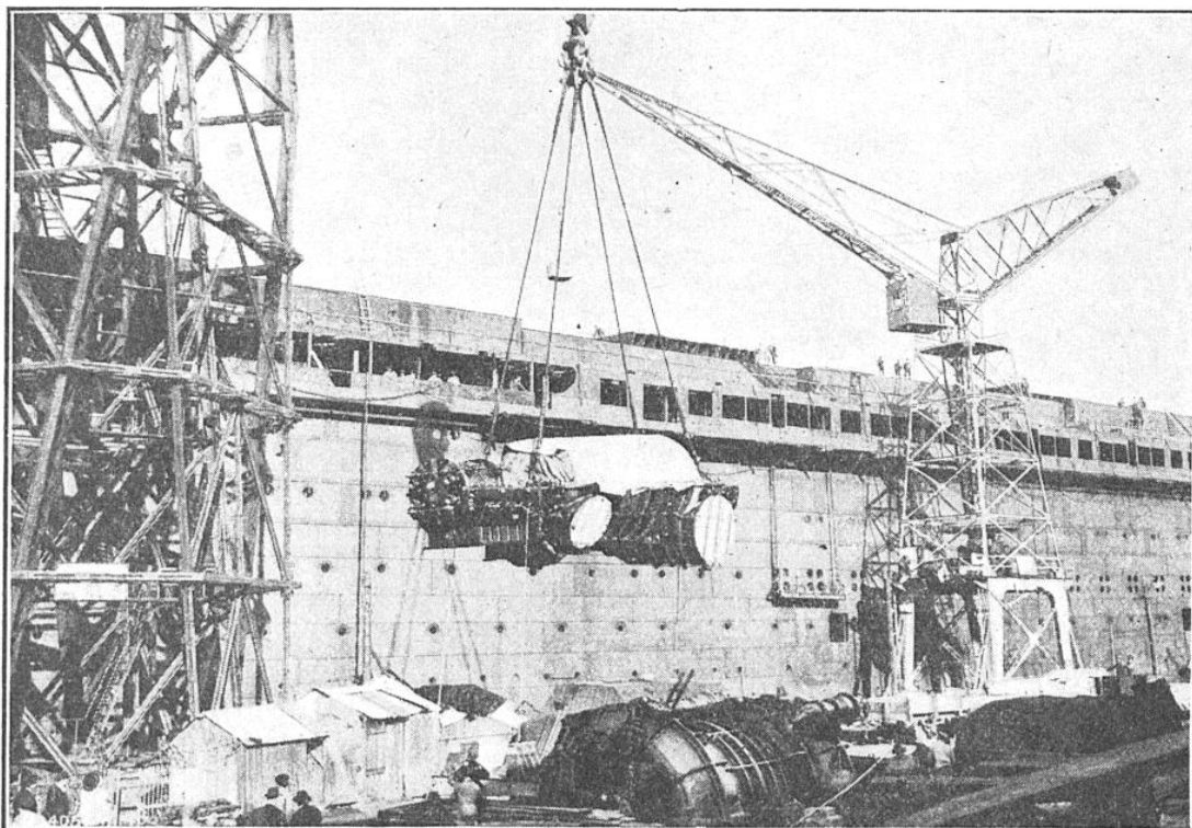
PREMIÈRE PHASE DE L'EMBARQUEMENT D'UNE TURBINE A BORD DU PAQUEBOT
