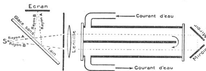
FIG. 4. — L'EFFET FRESNEL-FIZEAU
