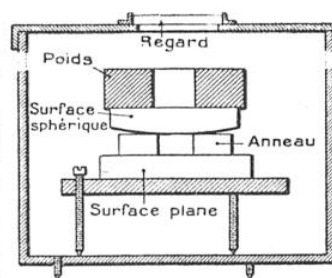
ÉTUVE DE L'APPAREIL DE M. ARNULF
