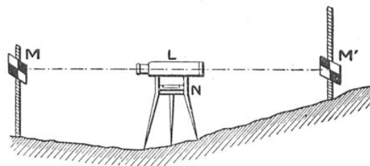
FIG. 6. — PRINCIPE DE LA MÉTHODE DE NIVELLEMENT GÉODÉSIQUE
