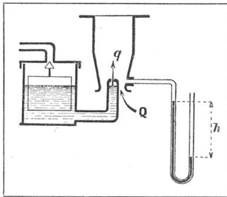
FIG. 3. — COUPE SCHÉMATIQUE D'UN CARBURATEUR A ESSENCE AVEC INDICATEUR DE DÉPRESSION
