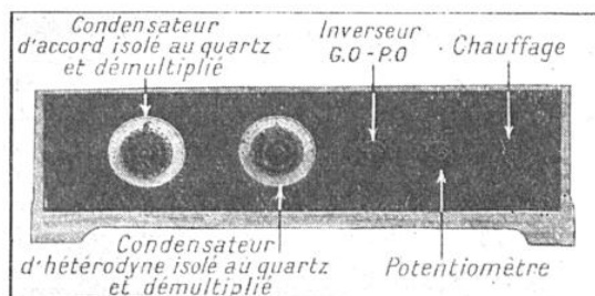
VUE EXTÉRIEURE DU « RÉBODYNE »
