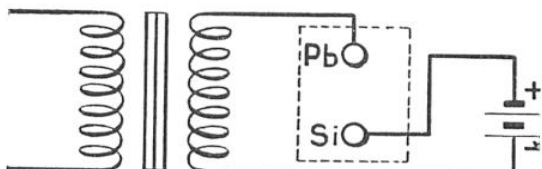
SCHÉMA DU BLOC DE CHAUFFAGE
