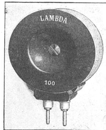
SELF EN NIDS D'ABEILLES PROTÉGÉE PAR DES JOUES D'ÉBONITE
