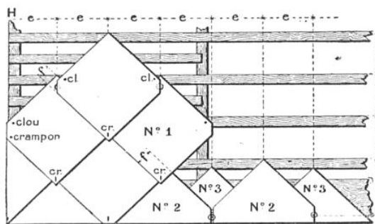
COUVERTURE A LA FRANÇAISE A COINS SUR-PLOMBANTS, AVEC TRIANGLES D'ÉGOUT POSÉS AVEC TAMPONS TEMPÊTE EN CUIVRE (ÉVERITE)
