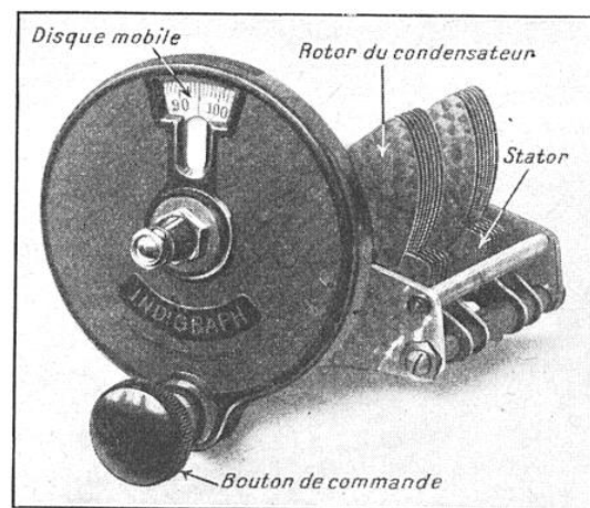
CONDENSATEUR VARIABLE POURVU DU CADRAN DÉMULTIPLICATEUR « INDIGRAPH »
