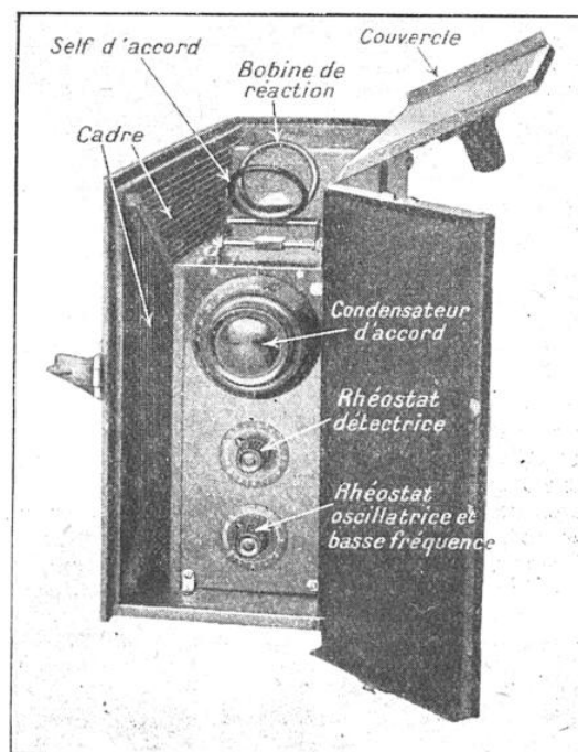
VUE INTÉRIEURE DU POSTE MALLETTE
