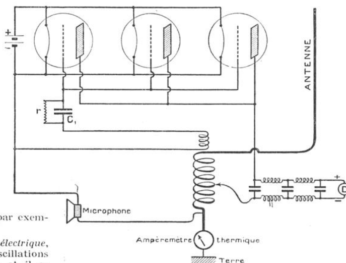
FIG. 21. — POSTE ÉMETTEUR A LAMPES
