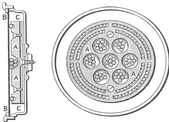
FIG. 1. — COUPE ET VUE EN PLAN D'UN MICROPHONE A, bloc de charbon creusé de cavités contenant de petites billes de charbon ; B, plaque de charbon circulaire et mince ; C, boîtier.
