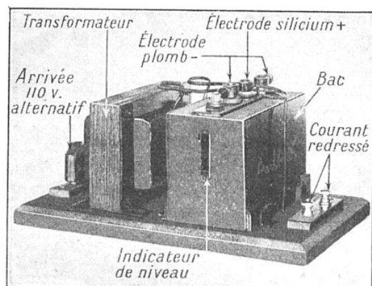
MODÈLE AJAX POUR LA RECHARGE DES ACCUS BASSE TENSION
