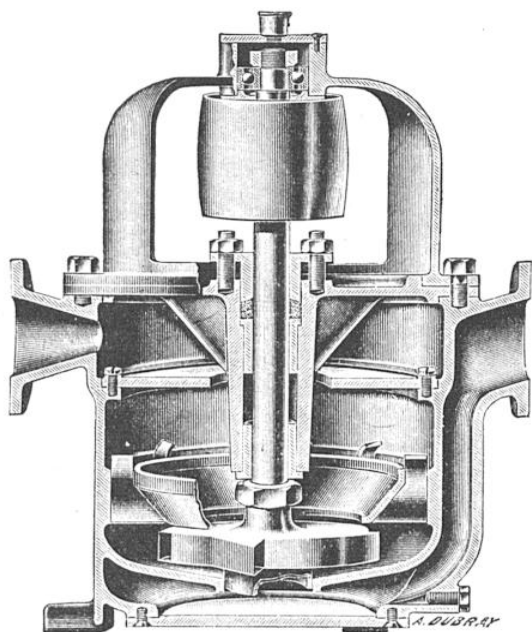
COUPE DE LA POMPE MAROGER
