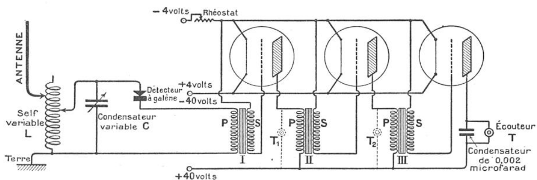
FIG. 12. — AMPLIFICATEUR A BASSE FRÉQUENCE ET A TRANSFORMATEURS
