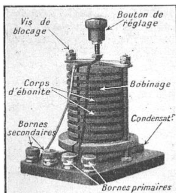
TRANSFORMATEUR GODY
