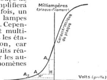
FIG. 14. — PRINCIPE DE LA DÉTECTION PAR LA LAMPE A TROIS ÉLECTRODES
