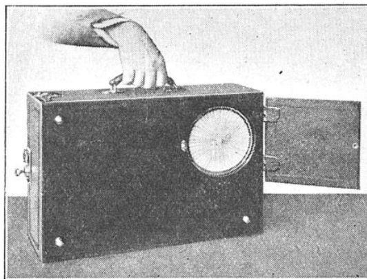
LE POSTE MALLETTE PRÊT POUR LE TRANSPORT Le haut-parleur est découvert
