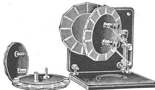
SUPPORTS DE SELF FOND DE PANIER La rotation se fait autour d'une charnière.
