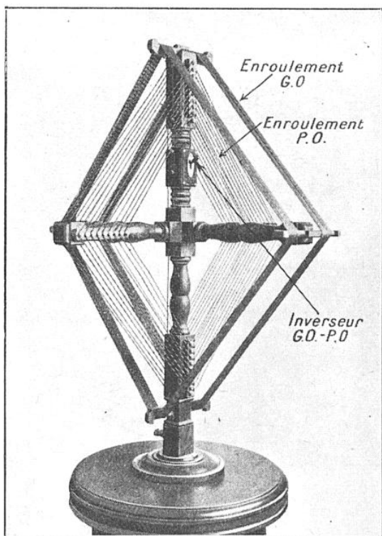
LE CADRE A DEUX ENROULEMENTS DU POSTE CHANGEUR DE FRÉQUENCE P. R. E. F. 9
