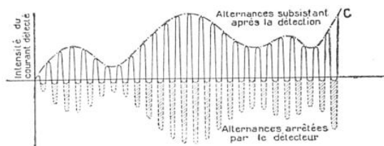
FIG. 7. — COURANT DÉTECTÉ
