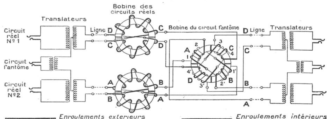
FIG. 9. — CHARGEMENT D'UNE « QUARTE » AU MOYEN DE TROIS BOBINES
