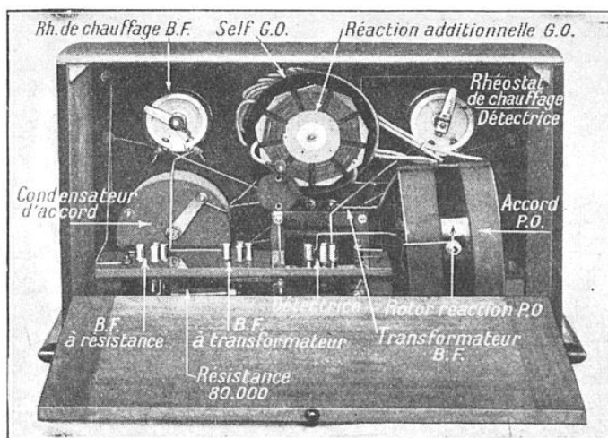
RÉCEPTEUR « MICRODYNE » A 3 LAMPES LEMOUZY
