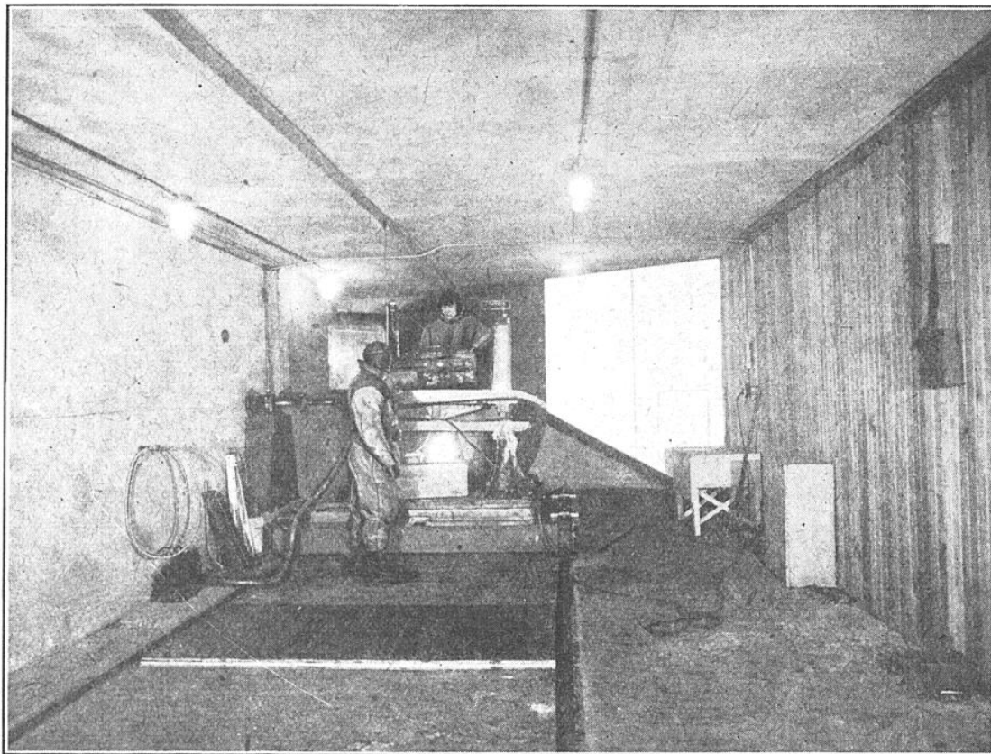
LES VOITURES SONT ESSAYÉES A LA CHAMBRE FROIDE (A 15° C. AU-DESSOUS DE ZÉRO) AUX LABORATOIRES DE LA « GENERAL MOTORS CO. »
