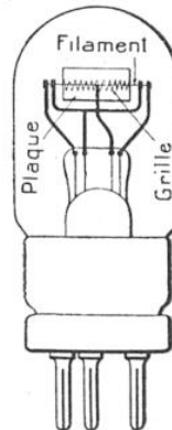
LAMPE A FAIBLE CONSOMMATION (6/100 e A) POUR AMPLIFICATION H. F.
