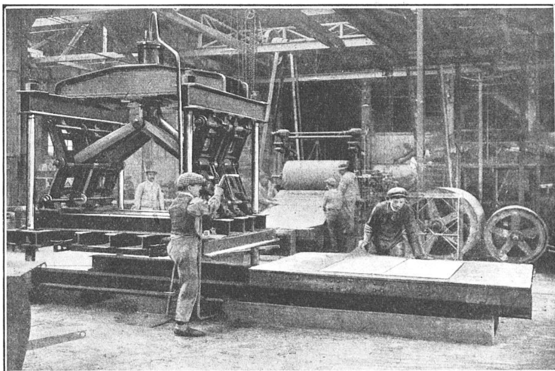
MACHINE A FABRIQUER L'ÉVERITE
