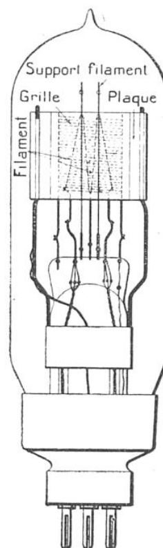
LAMPE POUR ÉMISSION « E. 5 » A PLAQUE DE MOLYBDÈNE
