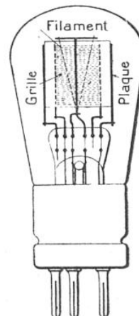
LAMPE « C. L. 164 » A FAIBLE CONSOMMATION (AMPLIFICATION A RÉSISTANCE)
