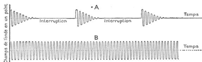
FIG. 4. — ONDES AMORTIES ET ONDES ENTRETENUES A, trains d'ondes amorties séparés par des interruptions ; B, ondes entretenues.
