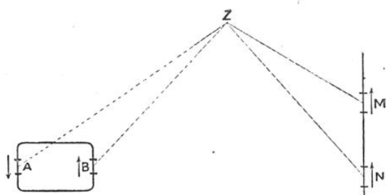
FIG. 20. — SUPÉRIORITÉ DE L'ANTENNE SUR UN CIRCUIT OSCILLANT FERMÉ.
