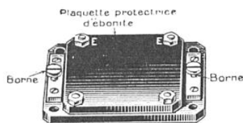
UN CONDENSATEUR FIXE A LAMES D'ÉTAIN ET DE MICA
