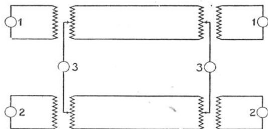
FIG. 7. - CIRCUIT RÉEL ET CIRCUIT FANTÔME, OU COMBINÉ
