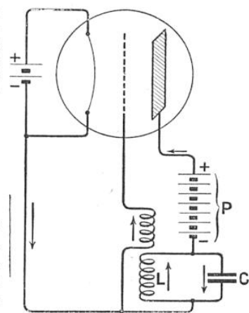
FIG. 19. — LAMPE GÉNÉRATRICE D'OSCILLATIONS ENTRETENUES
