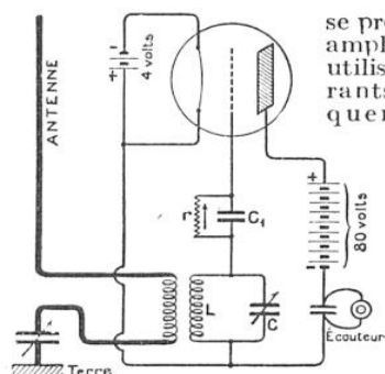
FIG. 15. — MONTAGE POUR UN AUTRE MODE DE DÉTECTION
