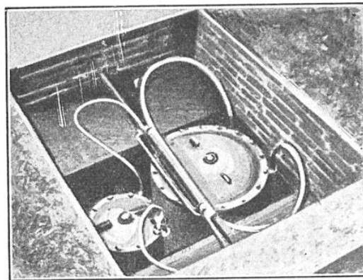
FIG. 6. — CHAMBRE A DEUX BOBINES PUPIN (CABLE DE LYON A SAINT-ÉTIENNE)
