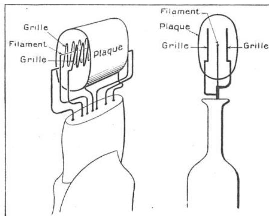
DESSIN MONTRANT LA DISPOSITION DES GRILLES ET DE LA PLAQUE
