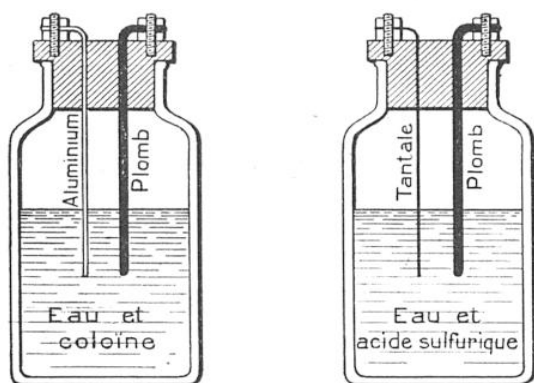
LES DEUX VALVES DU REDRESSEUR « C. R. E. J. » cesse de fournir la tension anodique et recharge automatiquement l'accumulateur.
