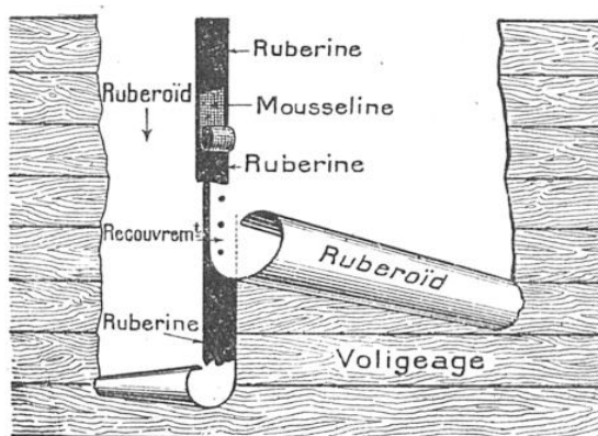
MÉTHODE DE POSE DU RUBÉROÏD SUR UNE TOITURE
