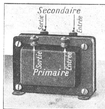
SUPER-TRANSFORMATEUR BARDON
