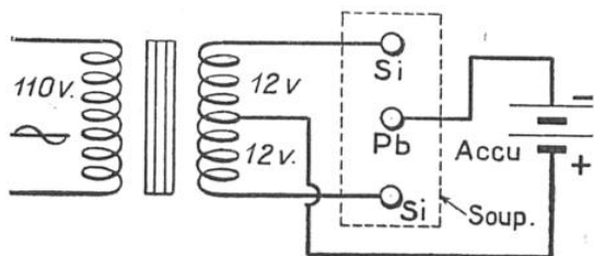
SCHÉMA DE LA RECHARGE DES ACCUS B. T.
