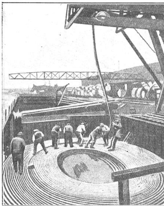
FIG. 10. — VUE DU CHARGEMENT EN PÉNICHES DU CÂBLE DE LA FIRME SIEMENS UND HALSKE. LA PORTION SUSPENDUE CORRESPOND A UN TRONÇON PUPINISÉ
