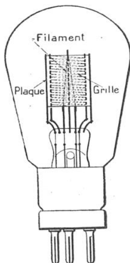
LAMPE « C. L. 975 » POUR AMPLIFICATION DE PUISSANCE (HAUT-PARLEURS D'EXTÉRIEUR)
