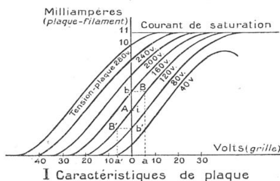
FIG. 11. — CARACTÉRISTIQUES DE PLAQUE ET DE GRILLE
