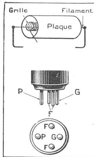
LA LAMPE A TROIS ÉLECTRODES
