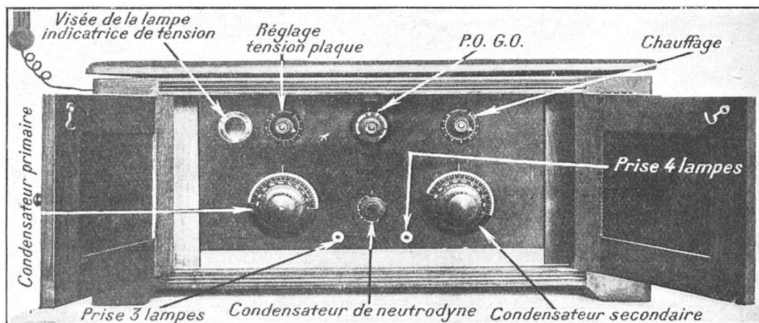
RÉCEPTEUR A ALIMENTATION DIRECTE «NORD-ALTERNA»
