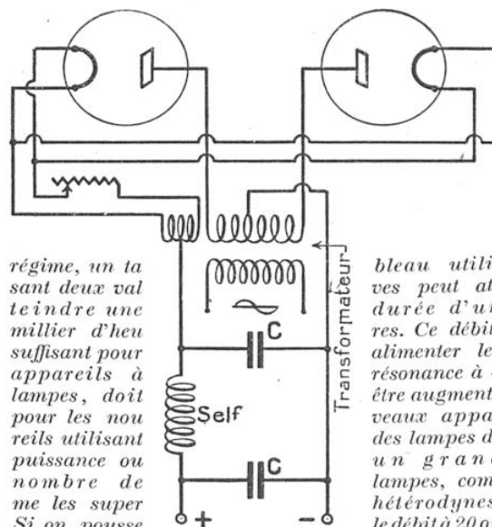
LES DEUX VALVES DU REDRESSEUR « C. R. E. J. » cesse de fournir la tension anodique et recharge automatiquement l'accumulateur.
