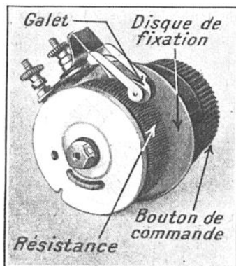
RHÉOSTAT DYNA
