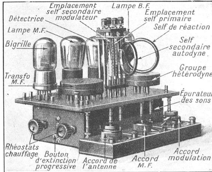
LE MICRODION-MODULATEUR HURM
