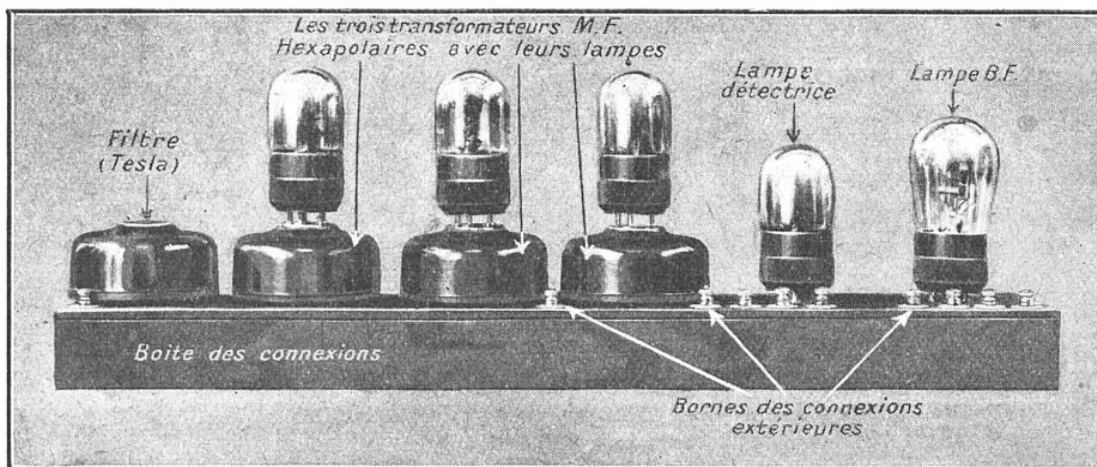
LE BLOC AMPLIFICATEUR COMPLET
