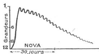
FIG. 7. — COURBE DE LUMIÈRE D'UNE ÉTOILE NOUVELLE AVEC SES OSCILLATIONS PÉRIODIQUES DANS LES PREMIÈRES SEMAINES DE SON APPARITION
