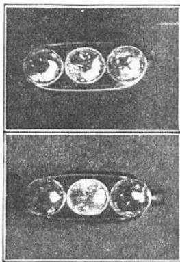
LES MÊMES DIAMANTS ÉCLAIRÉS PAR DE LA LUMIÈRE BLANCHE EN HAUT ET PAR DES RAYONS ULTRAVIO- LETS EN BAS
