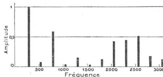
FIG. 6. — L'UT 3 DE LA CLARINETTE EST CONSTITUÉ DE VIBRATIONS SIMPLES FORT DIVERSES
