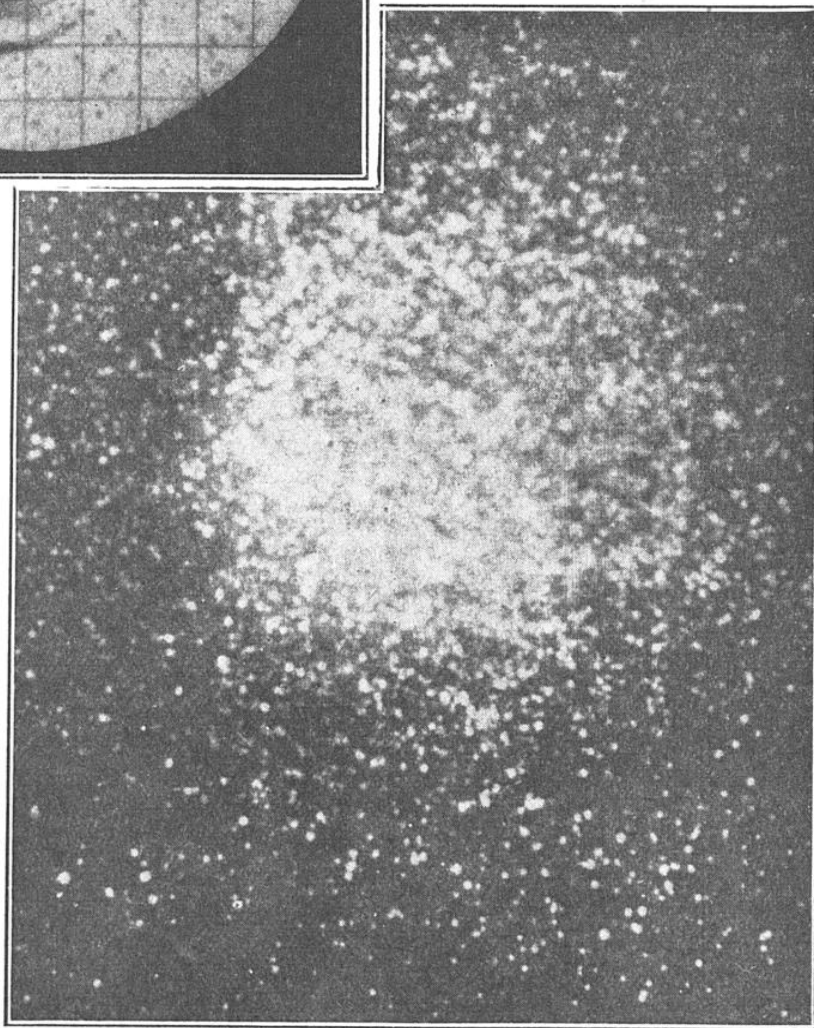
FIG. 4. — AMAS GLOBULAIRE DU CENTAURE, COMPRENANT PRÈS DE 100.000 SOLEILS, SITUÉ A 20.000 ANNÉES DE LUMIÈRE DE NOUS, LE PLUS RAPPROCHÉ DES AMAS GLOBULAIRES
