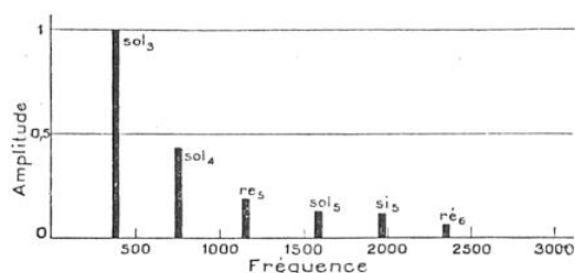
FIG. 5. — AMPLITUDES DES VIBRATIONS SIMPLES COMPOSANT LE SOL 3 DU VIOLON
