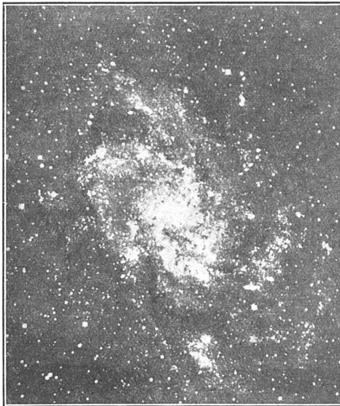
FIG. 10. — NÉBULEUSE SPIRALE DU TRIANGLE DISTANTE DE PRÈS D'UN MILLION D'ANNÉES DE LUMIÈRE. REMARQUER LES NOMBREUSES NODOSITÉS NÉBULEUSES OU STELLAIRES DANS LES SPIRES
