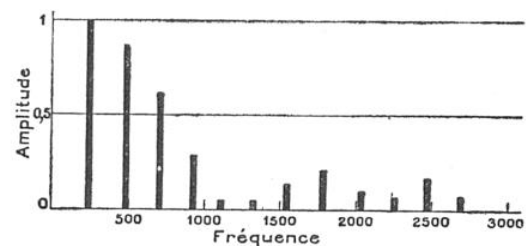
FIG. 8. — LA VOIX HUMAINE ( LA_2 ) EST TRÈS RICHE EN HARMONIQUES
