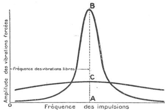
FIG. 9. — COURBE DE RÉSONANCE MONTRANT LES AMPLITUDES DU MOUVEMENT VIBRATOIRE D'UN CORPS ÉLASTIQUE POUR DIVERSES FRÉQUENCES D'IMPULSIONS AGISSANT SUR LUI
