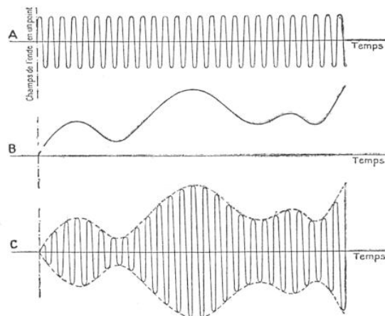
FIG. 6. — ONDES ÉLECTROMAGNÉTIQUES ET ONDES SONORES
