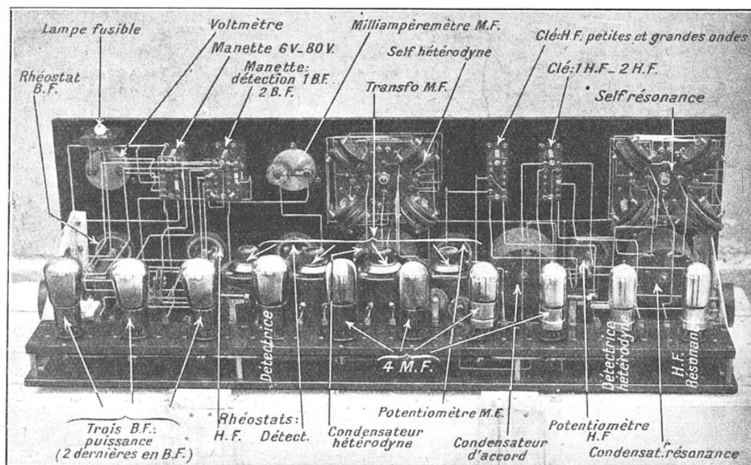
SUPERHÉTÉRODYNE 10 LAMPES RADIO-L. L.
