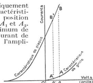
FIG. 16. — PRINCIPE DU MONTAGE PRÉCÉDENT
