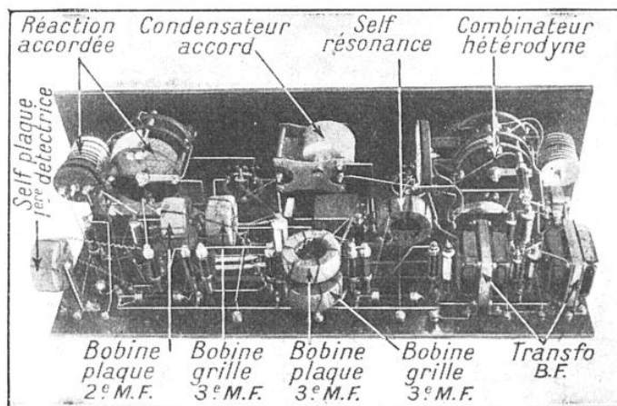
VUE INTÉRIEURE D'UN POSTE ULTRA-OSCILLATEUR A 10 LAMPES «VITUS»
