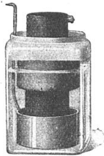
PILE FÉRY SUPER 3
