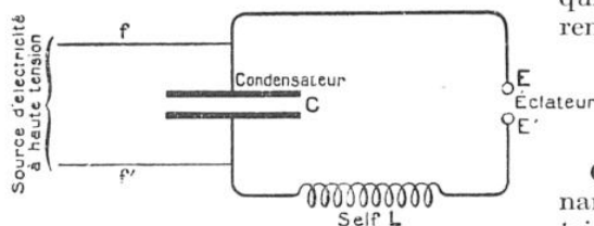
FIG. 1. — CE QU'ON ENTEND PAR CIRCUIT OSCILLANT
