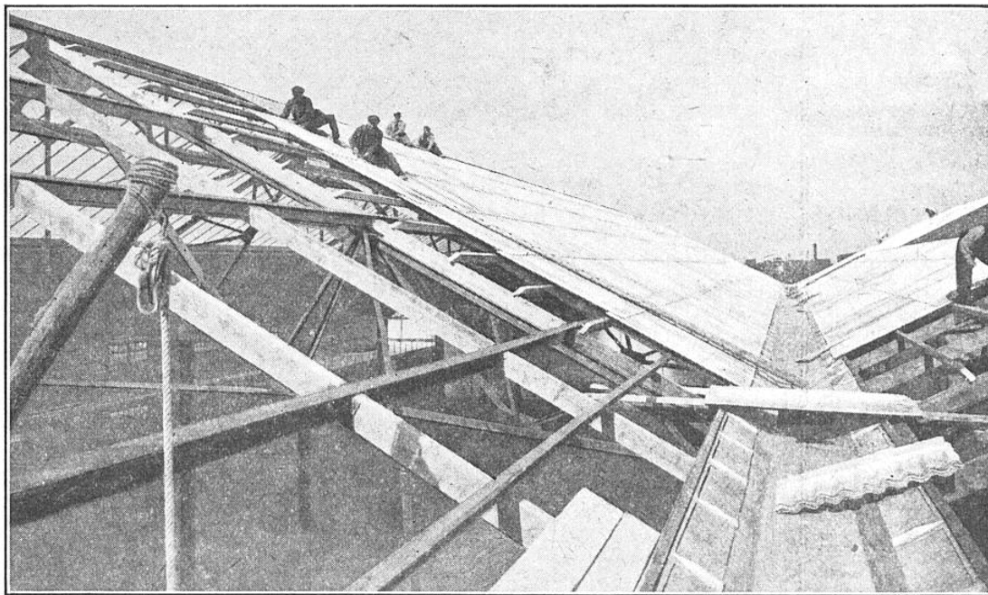
LA TOITURE DE BATIMENTS RECOUVERTS D'OURALITHE On remarque la légèreté de la charpente.
