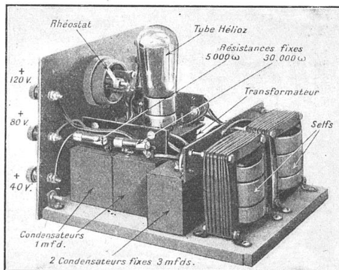
LE « BLOC HELIOR », VUE INTÉRIEURE
