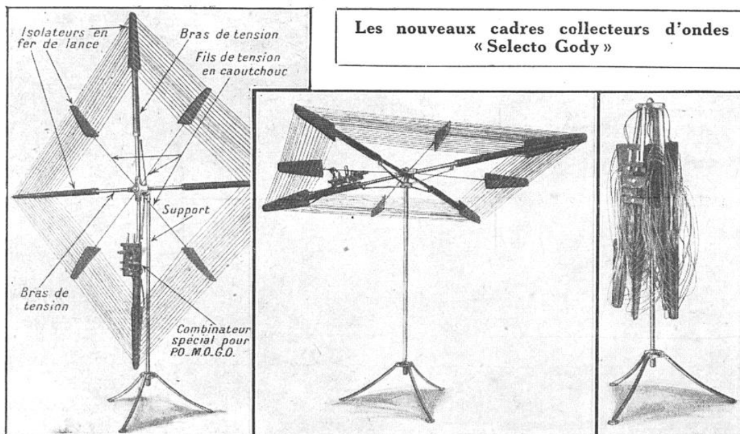
LE CADRE « PARAPLUIE » : A GAUCHE, DISPOSÉ VERTICALEMENT ; AU MILIEU, DISPOSÉ HORIZONTALEMENT ; A DROITE, REPLIÉ
