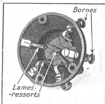
SUPPORT DYNA POUR LAMPES BIGRILLES
