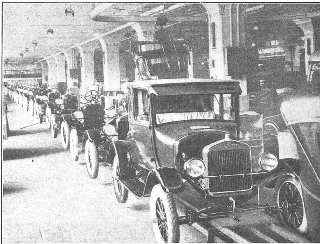
UNE LIGNE D'ASSEMBLAGE CHEZ FORD (DETROIT)
