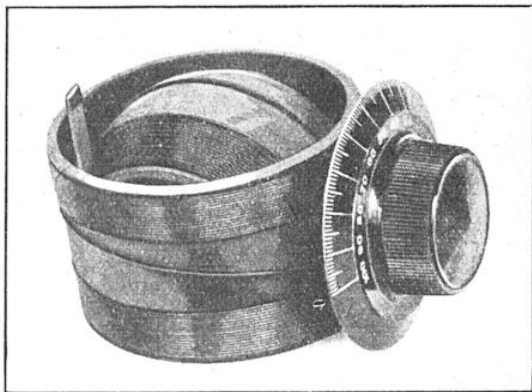
VARIOMÈTRE A BOBINE INTÉRIEURE SPHÉRIQUE, CONSTRUCTION LEMOUZY
