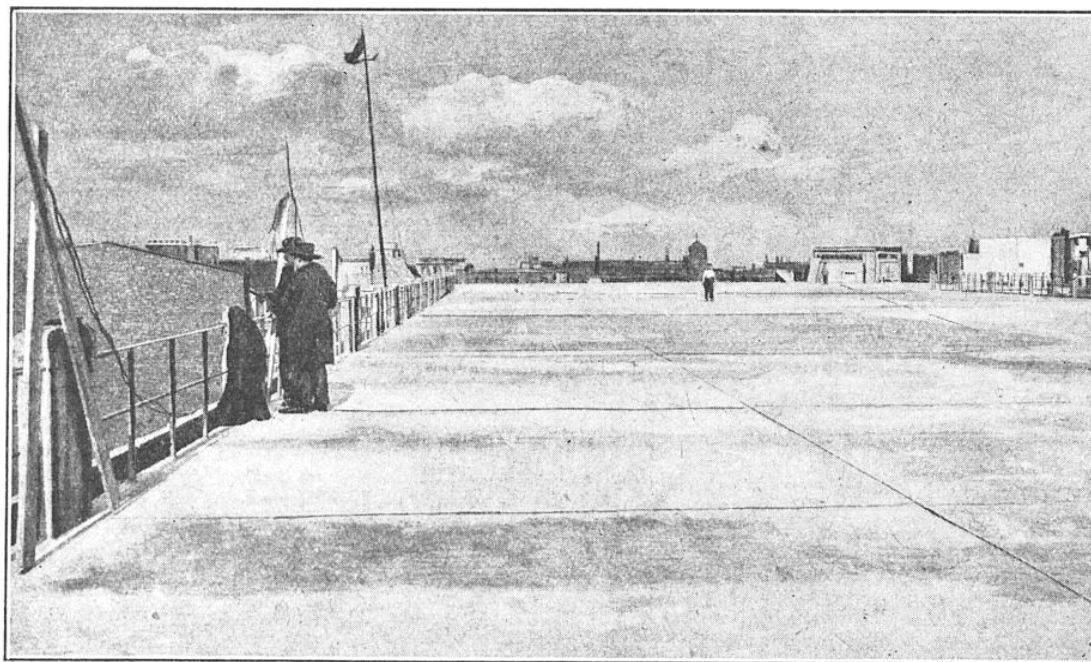
TERRASSE EN BÉTON ARMÉ ENDUITE AU COUVRANEUF
