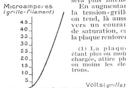
II Caractéristique de grille
