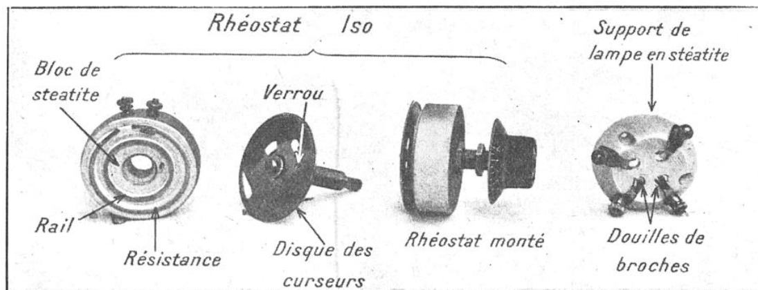
RHÉOSTAT ET SUPPORT DE LAMPE « ISO »
