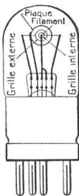
BIGRILLE « D. G. » AMPLIFICATRICE ET DÉTECTRICE FAIBLE TENSION PLAQUE
