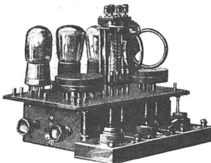
Microdion-Modulateur MM 4
