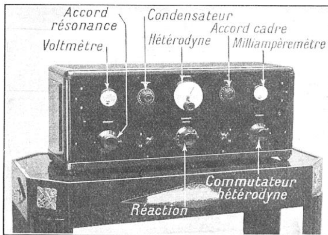
VUE EXTÉRIEURE D'UN POSTE « ULTRA-OSCILLATEUR » A 10 LAMPES VITUS
