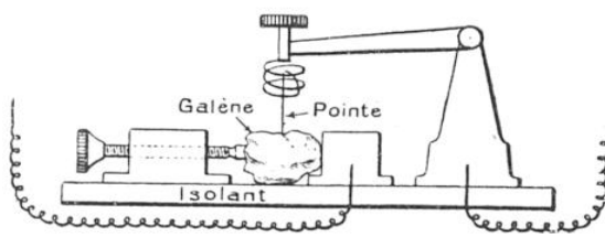
FIG. 8. — DÉTECTEUR A GALÈNE (SULFURE DE PLOMB)
