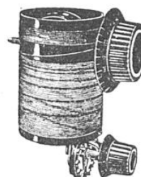
Variocoupleur B.. C.. 468 commuté
