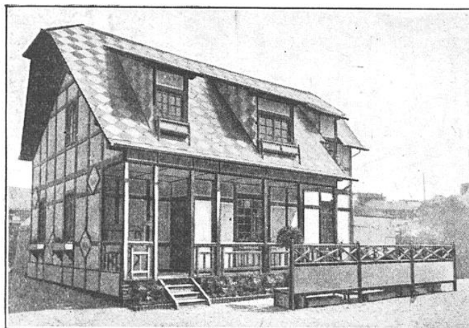
CHALET NORMAND EXÉCUTÉ EN ÉVERITE POUR LA FOIRE DE PARIS
