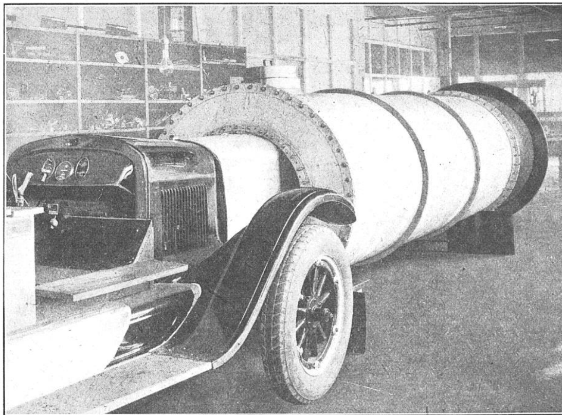
ESSAI DES RADIATEURS AU TUNNEL (CHEVROLET)
