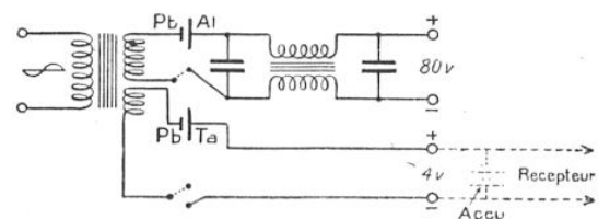
SCHEMA DES CONNEXIONS
