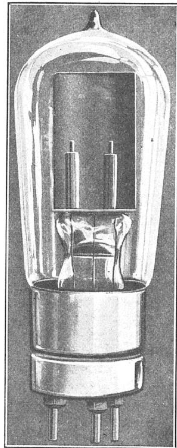
COUPE D'UN TUBE « HELIOR » SANS FILAMENT
