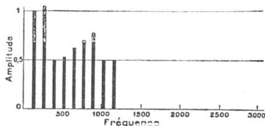
FIG. 7. — LE TROMBONE ( UT_2 ) DONNE DES SONS SUPÉRIEURS TRÈS DÉVELOPPÉS
