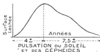
FIG. 8. — COURBE DE LA PULSATION UNDÉCENNALE DU SOLEIL. MESURÉE PAR LA SURFACE DES TACHES
