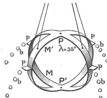
FIG. 9. — EXPÉRIENCE DE LA SPHÈRE ÉLASTIQUE ENTRANT EN PULSATION PAR DES CHOC SUR LA RÉGION POLAIRE « P ». LA PULSATION RENFLANT PÉRIODIQUEMENT L'ÉQUATEUR EN CHASSE LES BOULES « B » PLACÉES SUR LES PLATEAUX « p », COMME LA PULSATION DU PROTOSOLEIL A FAIT ÉMETTRE À SON ÉQUATEUR LES NAPPES PLANÉTAIRES
