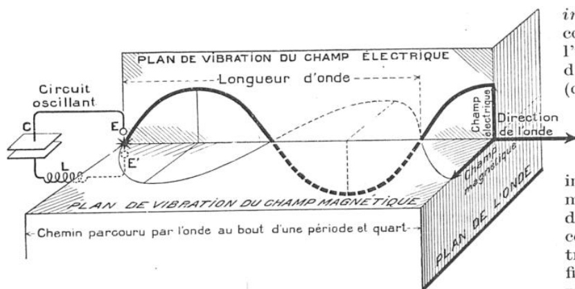
FIG. 2. — CONSTITUTION D'UNE ONDE ÉLECTROMAGNÉTIQUE
