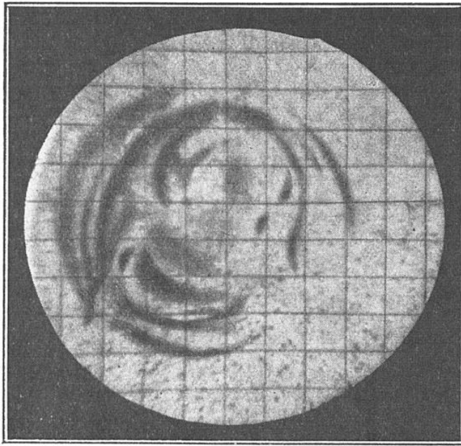
FIG. 3. — PHOTOGRAPHIE (EN NÉGATIF) DES NAPPES NÉBULEUSES ISSUES DE LA NOVA DE PERSÉE 1901 ET S'EN ÉCARTANT A GRANDE VITESSE (SEPTEMBRE 1901)
