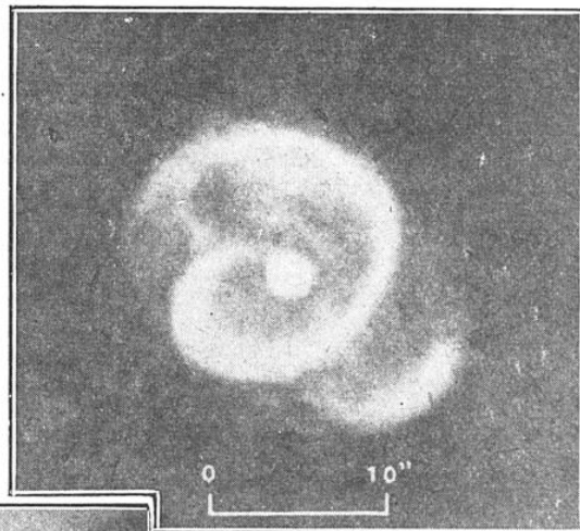
FIG. 6. — NÉBULEUSE EN HÉLICE (NGC 6543), PHOTOGRAPHIÉE PAR CURTIS
