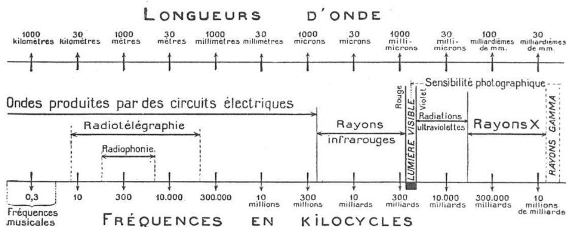
FIG. 3. — LES DIFFÉRENTES SORTES D'ONDES ÉLECTROMAGNÉTIQUES
