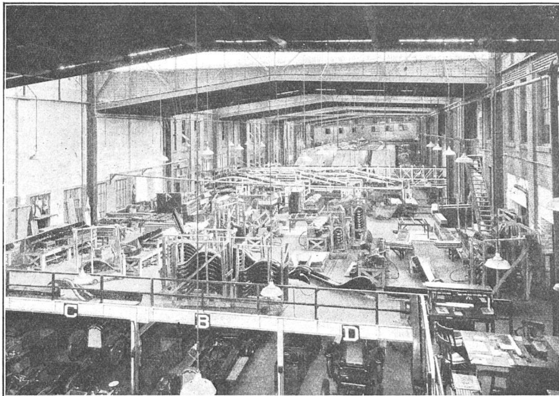
LES TROIS LIGNES DE MONTAGE AUX USINES BUICK
