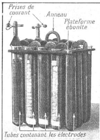
VUE INTÉRIEURE DE LA BATTERIE
