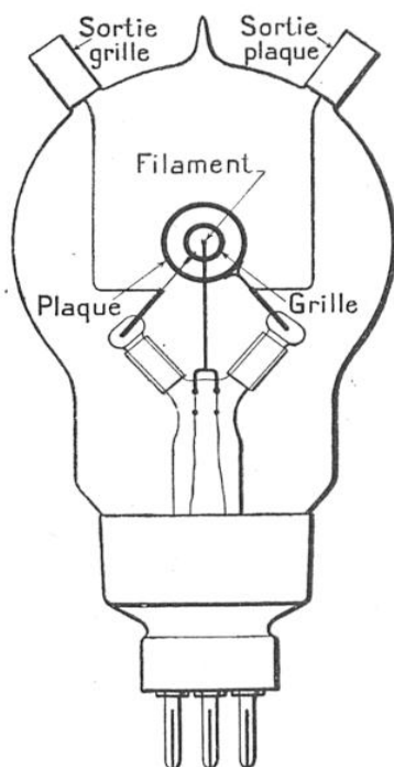
LAMPE « E. 4 M. » A PLAQUE DE MOLYBDÈNE POUR ÉMISSION SUR ONDES COURTES
