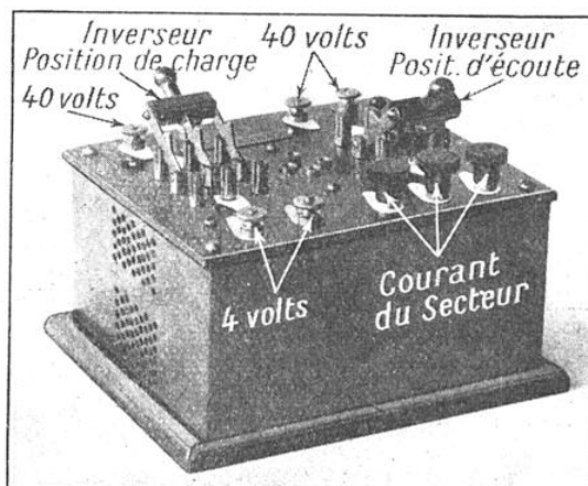
VUE EXTÉRIEURE DU REDRESSEUR « FARAD »
