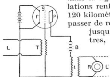
FIG. 5. - LAMPE TRIODE MONTÉE EN AMPLIFICATEUR
