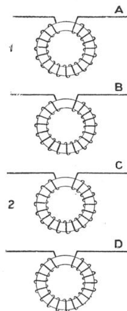
FIG. 8. - CHARGEMENT D'UNE « QUARTE » AVEC DES BOBINES UNIFILAIRES
