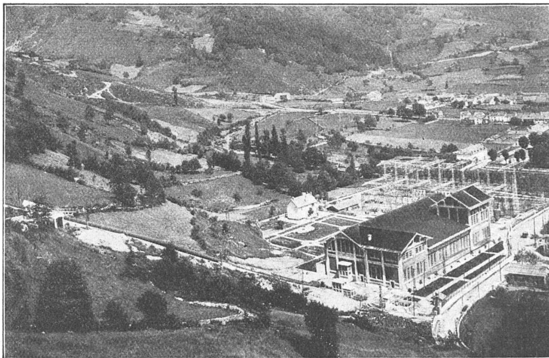
VUE D'ENSEMBLE DE L'USINE DU HOURAT (VALLÉE D'OSSAU), D'UNE PUISSANCE TOTALE DE 50.000 CH. EN ARRIÈRE DE L'USINE, LE POSTE DE DÉPART A 150.000 VOLTS
