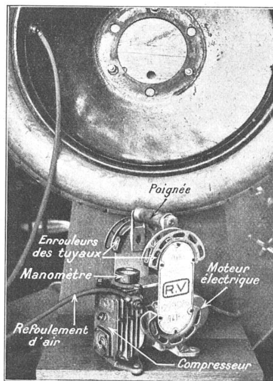
FIG. 21. - COMPRESSEUR D'AIR « RENÉ VOLET » POUR GONFLER LES PNEUMATIQUES
