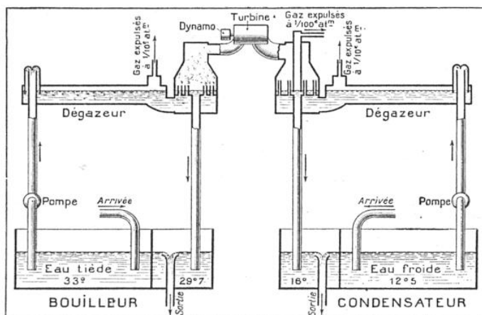
SCHÉMA GÉNÉRAL DE L'INSTALLATION CLAUDE-BOUCHEROT
