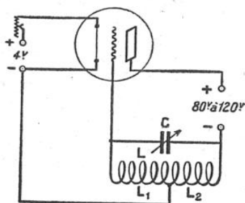
FIG. 1. - SCHÉMA DE MONTAGE DE L'HÉTÉRODYNE
