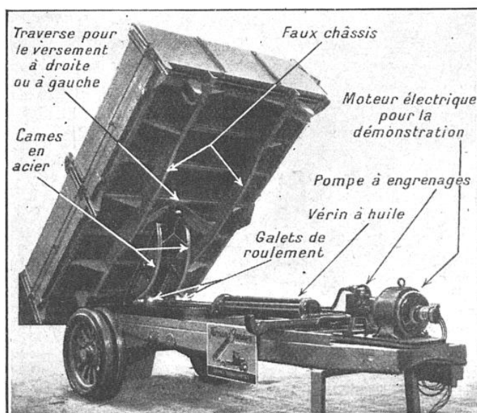
FIG. 24. — SYSTÈME BASCULEUR « FERNAND GENÈVE »
