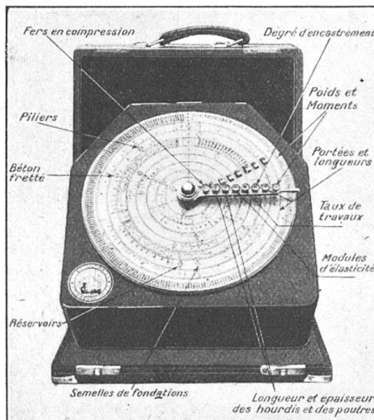
FIG. 25. — LA MACHINE « WASHINGTON »
