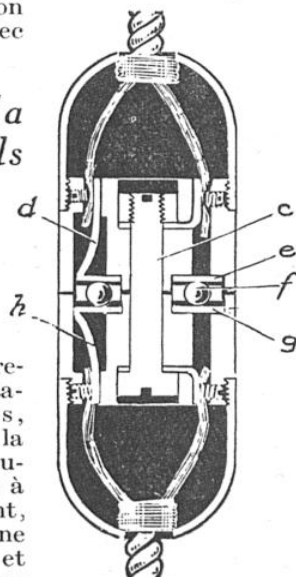
LE « ROTOCONTACT »
