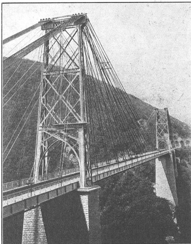
DEUX OUVRAGES D'ART DE LA PREMIÈRE LIGNE TRANS-PYRÉNÉENNE A VOIE ÉTROITE DE UN MÈTRE : DE VILLE-FRANCHE A BOURG-MADAME
