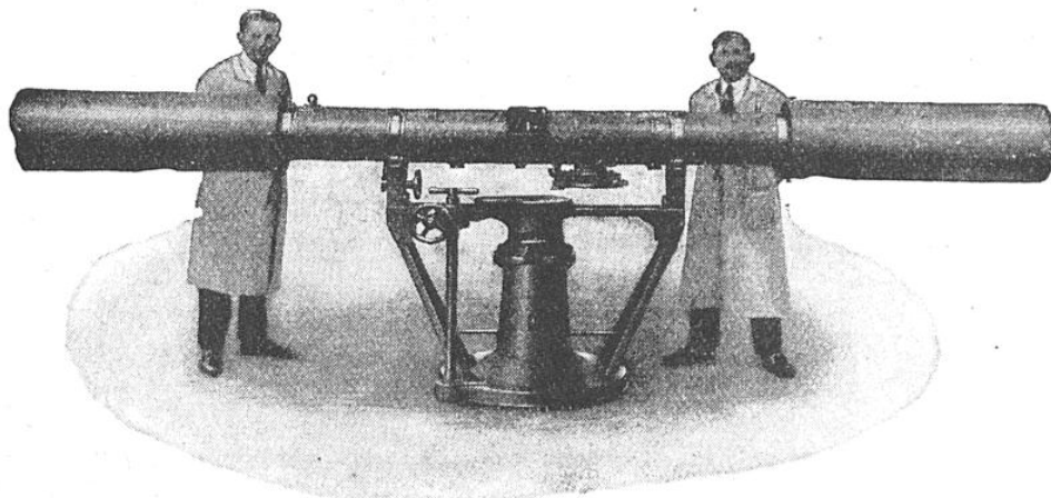
Télémètre à coïncidence de 4 mètres de base, type « Marine », armant les croiseurs de 8.000 tonnes
