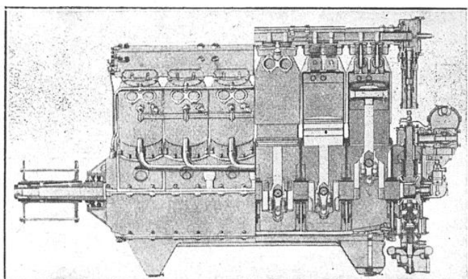
MOTEUR BREITFELD-DANEK DE 500-760 CH
