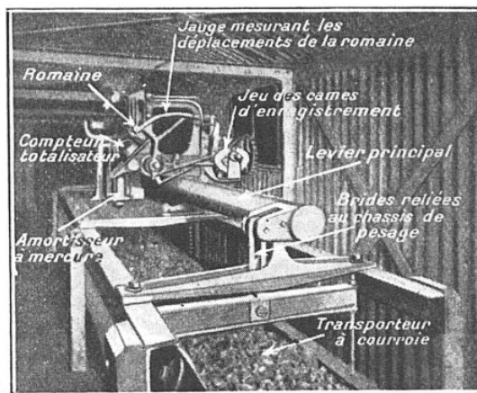
FIG. 14. - BASCULE AUTOMATIQUE « DENISON »
