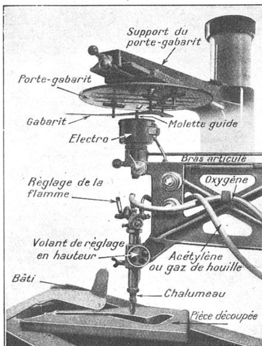
FIG. 22. — NOUVELLE MACHINE A DÉCOUPER LES TUBES « S. A. F. »
