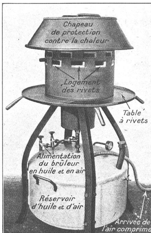
FIG. 16. — FOUR A CHAUFFER LES RIVETS « ELREY »
