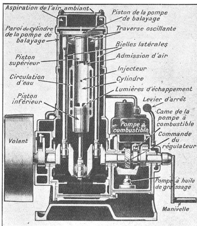
FIG. 17. — LE NOUVEAU MOTEUR « PEUGEOT » (LICENCE JUNKERS)
