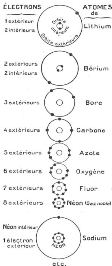
REPRÉSENTATION SCHEMATIQUE DU NOMBRE ET DE LA POSITION RELATIVE DES ÉLECTRONS DANS DIVERS ÉLÉMENTS
