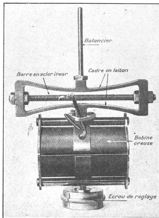
FIG. 10. — LE BALANCIER COMPENSATEUR
