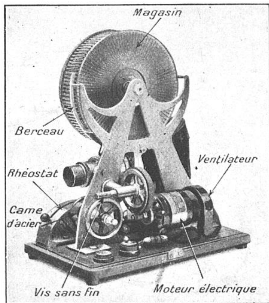
L'APPAREIL DE PROJECTION LUMINEUSE VU DU COTÉ DU MOTEUR
