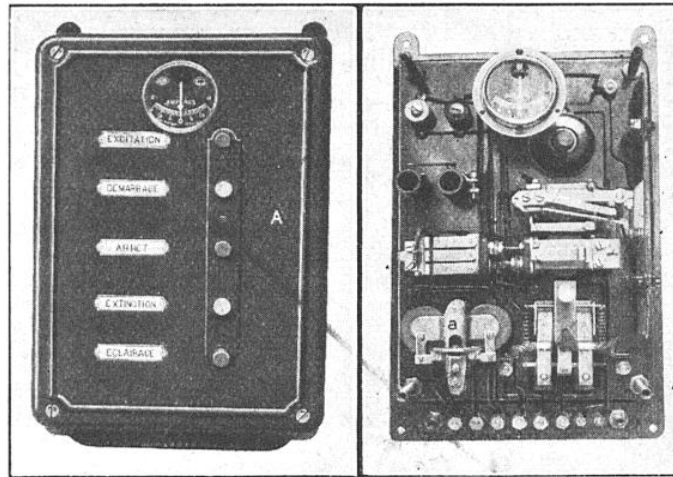
FIG. 3. — LE TABLEAU, VUES EXTÉRIEURE ET INTÉRIEURE A, régulateur E. H. R.
