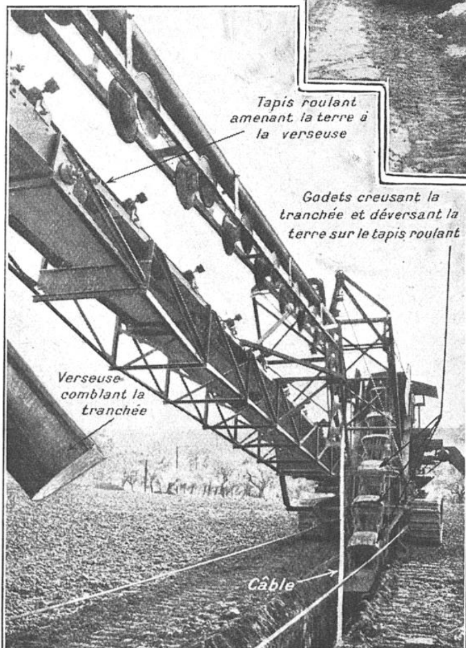
VUE PARTIELLE DE LA MACHINE PRISE DE L'ARRIÈRE
