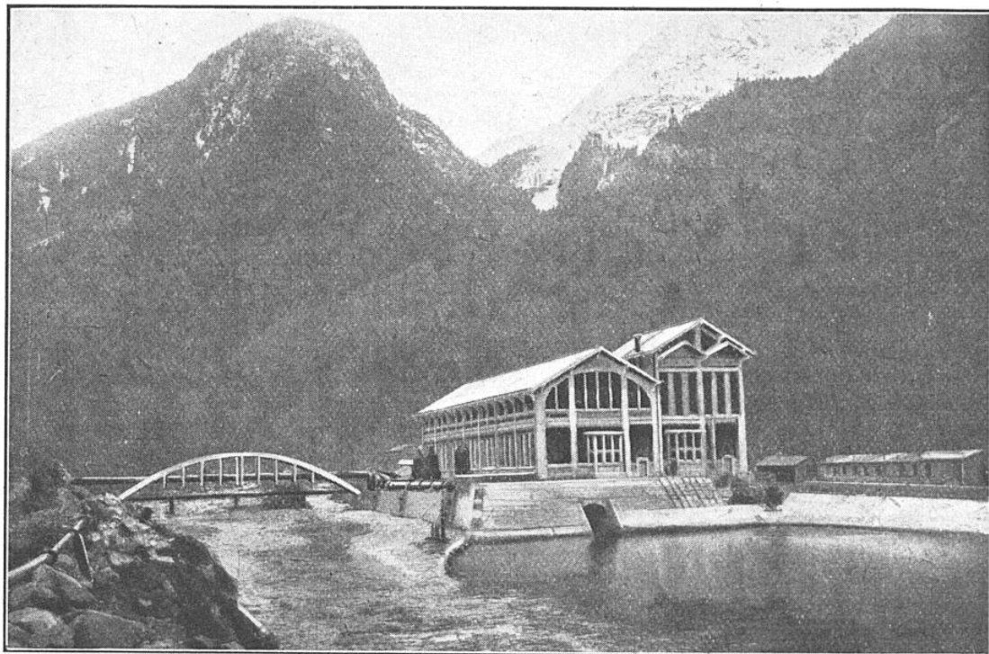
VUE GÉNÉRALE DE L'USINE DE MIÉGEBAT (VALLÉE D'OSSAU), QUI COMPORTE CINQ TURBINES PELTON DONNANT UNE PUISSANCE DE 50.000 CH SOUS UNE CHUTE DE 396 MÈTRES
