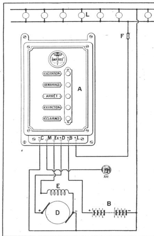
FIG. 4. — SCHÉMA DE L'INSTALLATION A, tableau ; B, accumulateurs ; D, dynamo ; L, lampes ; m, contact d'arrêt du moteur qui agit quand la batterie est chargée.
