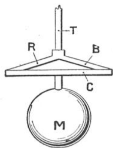
FIG. 8. — PRINCIPE DU COMPENSATEUR DE M. FAVRE BULLE T, tige du pendule ; RBC, triangle ; M, masse pendulaire.
