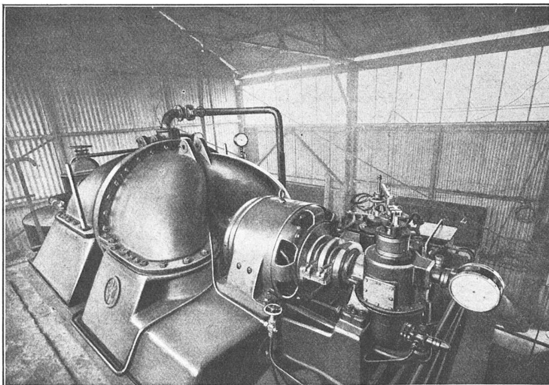
LE GROUPE TURBO-GÉNÉRATEUR DE 50 KILOWATTS
