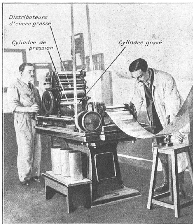
ENSEMBLE DE LA MACHINE A IMPRIMER (DÉPOT DE L'ENCRE GRASSE SUR LE FILM).
