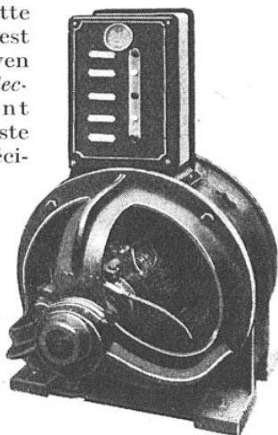
FIG. 2. — LA DYNAMO ET SON RÉGULATEUR E. H. R. PLACÉ DANS UN COFFRET
