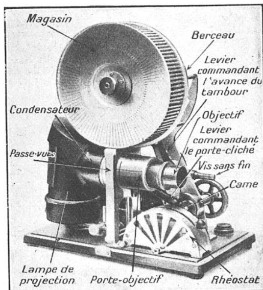
PHOTOGRAPHIE DE L'APPAREIL MONTRANT LE PASSE-VUES ET LE DISPOSITIF DE PROJECTION
