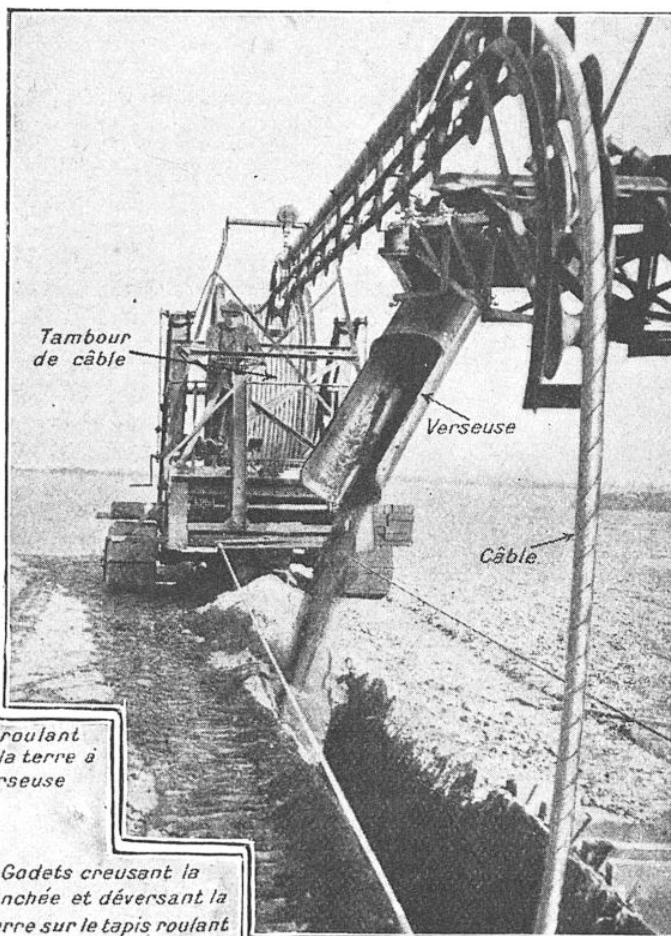
VUE PARTIELLE DE LA MACHINE PRISE DE L'AVANT ET MONTRANT LE DÉVERSEMENT DE LA TERRE
