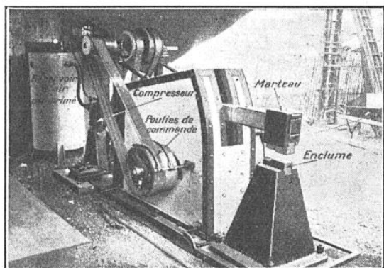
FIG. 15. — MARTEAU MÉCANIQUE « RECORD »
