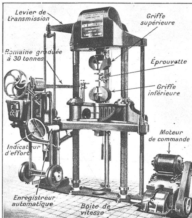
FIG. 13. — MACHINE D'ESSAIS UNIVERSELLE « FALCOT ET CHARPENTIER », TYPE VERTICAL
