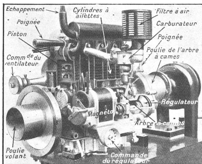
FIG. 20. — LE POLYMOTEUR
