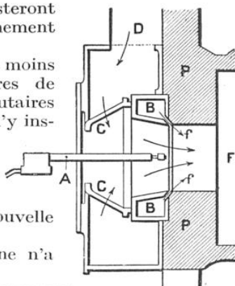
BRÛLEUR MIXTE «PEABODY» POUR LA CHAUFFE AU MAZOUT ET AU CHARBON PULVÉRISÉ
