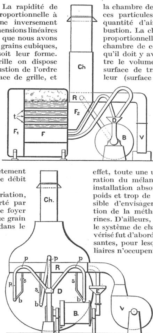
SCHÉMA D'UNE INSTALLATION DE CHAUFFE AU CHARBON PULVÉRISÉ. EN HAUT, COUPE LONGITUDINALE ; EN BAS, VUE DE FACE
