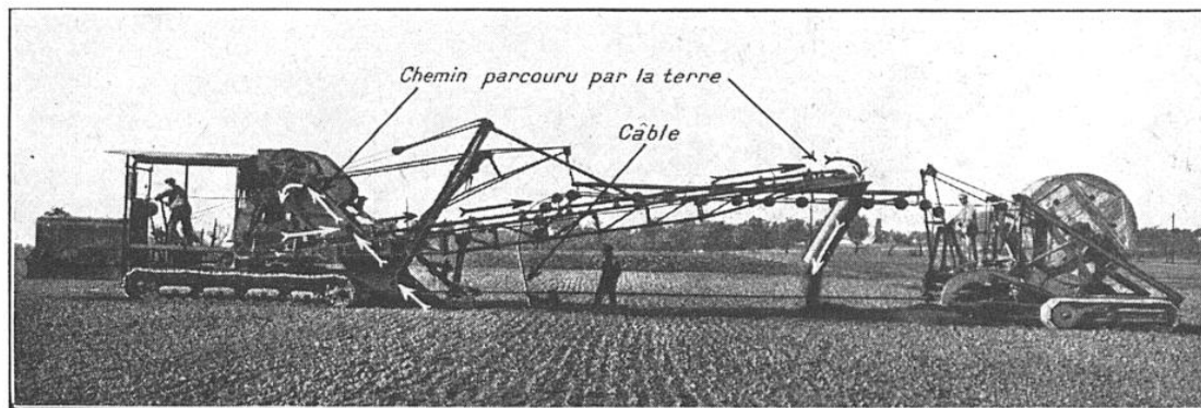
VUE D'ENSEMBLE DE LA MACHINE A POSER LES CABLES ÉLECTRIQUES
