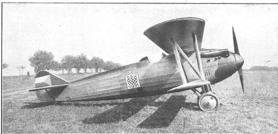
AVION DE CHASSE LETOV « S.-20 », ÉQUIPÉ AVEC UN MOTEUR HISPANO DE 300 CH ET FOURNI AUX ARMÉES LITHUANIENNE ET YOUGOSLAVE
