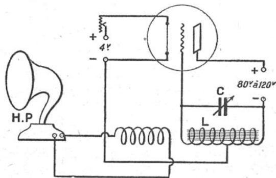
FIG. 2. — SCHÉMA DE MONTAGE DU PRODUCTEUR ÉLECTROMAGNÉTIQUE D'ONDES SONORES
