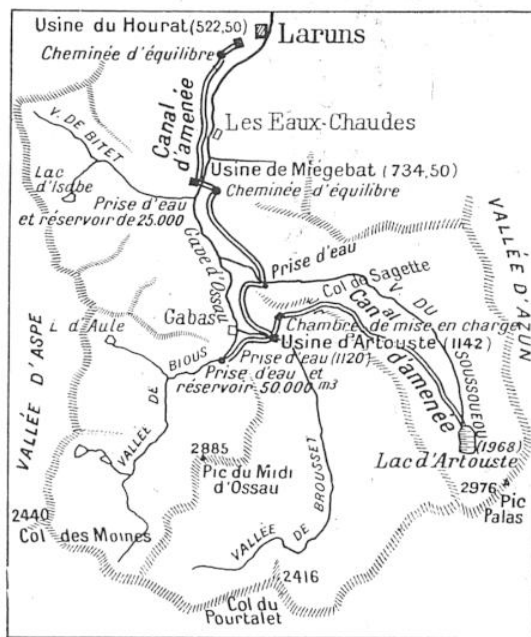
CARTE DE LA VALLÉE D'OSSAU MONTRANT LA RÉPARTITION DES CENTRALES ÉLECTRIQUES
