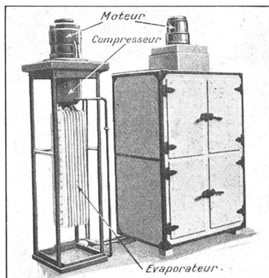
FIG. 6. - LA MACHINE FRIGORIFIQUE « BOREAS »
