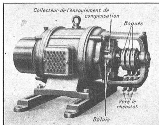
FIG. 2. — MOTEUR ASYNCHRONE AUTOCOMPENSÉ DE LA SOCIÉTÉ ALSACIENNE DE CONSTRUCTIONS MÉCANIQUES
