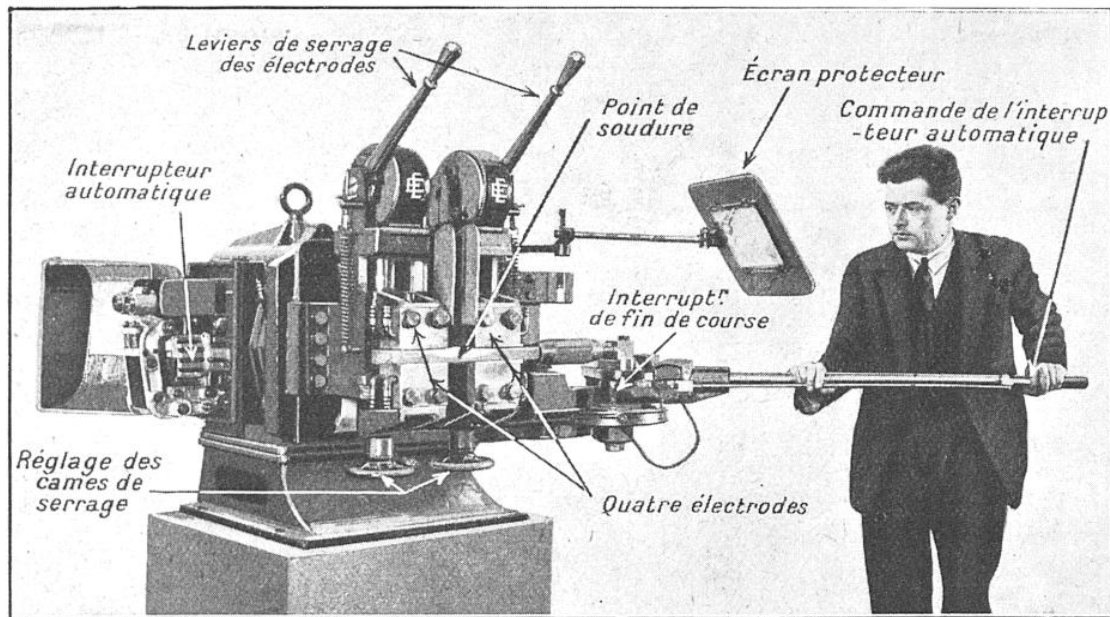
FIG. 3. — LA MACHINE ÉLECTRIQUE À SOUDER PAR BOUTS DE L'ÉLECTRO-OUTILLAGE
