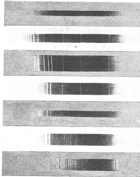
TYPES DE SPECTRES D'ÉTOILES (Observatoire de Harvard College, Cambridge U. S. A.)
