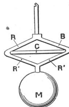
FIG. 9. — DEUX TRIANGLES DE LAITON RBR'R' ACCOLÉS PAR LEUR BASE C EN INVAR, DONNENT L'EFFET DE COMPENSATION
