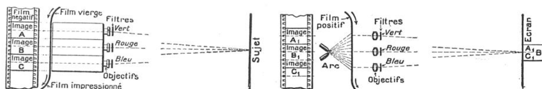
LE PRINCIPE DU CINÉMA EN COULEURS DES FRÈRES GAUMONT
