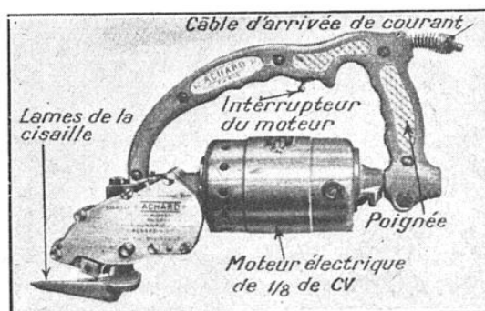
FIG. 12. — LA CISAILLE « ACHARD »
