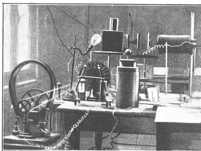
DISPOSITIF UTILISÉ PAR M. A. NODON À LA SORBONNE, EN 1901, POUR LA DÉCOUVERTE DE RAYONS X DE GRANDE LONGUEUR D'ONDE
