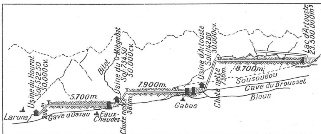
SCHEMA D'UTILISATION DES EAUX DEPUIS LE LAC D'ARTOUSTE JUSQU'À L'USINE DU HOURAT
