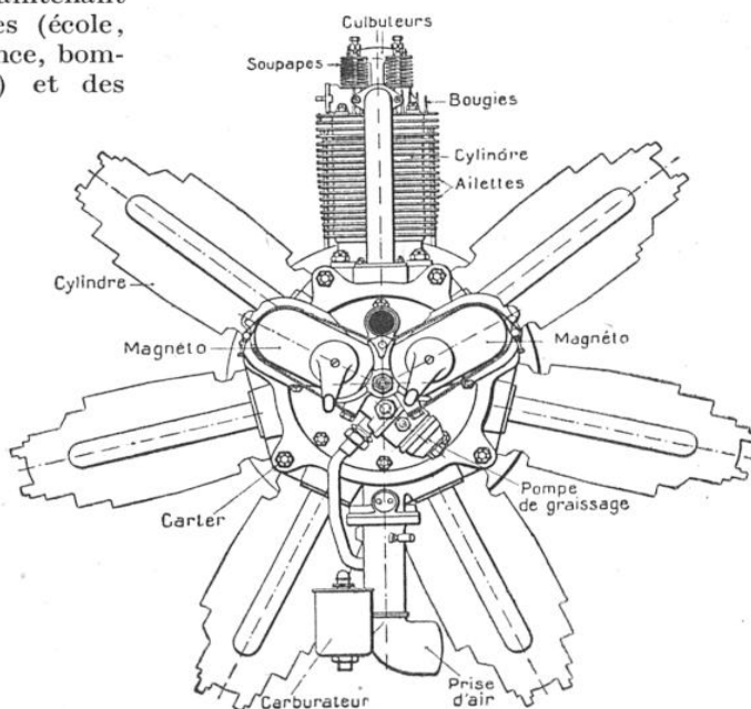
MOTEUR D'AVIATION WALTER 85 A REFROIDISSEMENT PAR AIR, TYPE N.-2, VU DE L'ARRIÈRE
