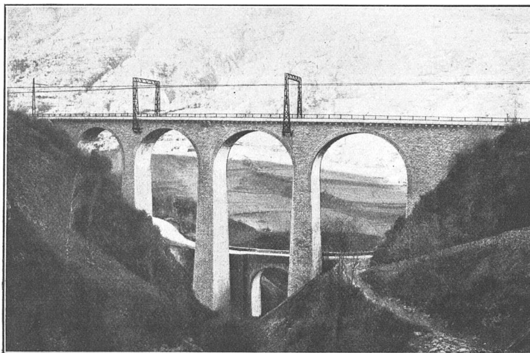
VIADUC DE « L'ARNOUSE » SUR LA LIGNE DE BEDOUS A LA FRONTIÈRE
