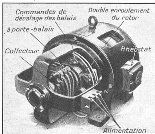
FIG. 1. — MOTEUR AUTOCOMPENSÉ DE LA SOCIÉTÉ DE CONSTRUCTIONS ÉLECTRIQUES DE JEUMONT
