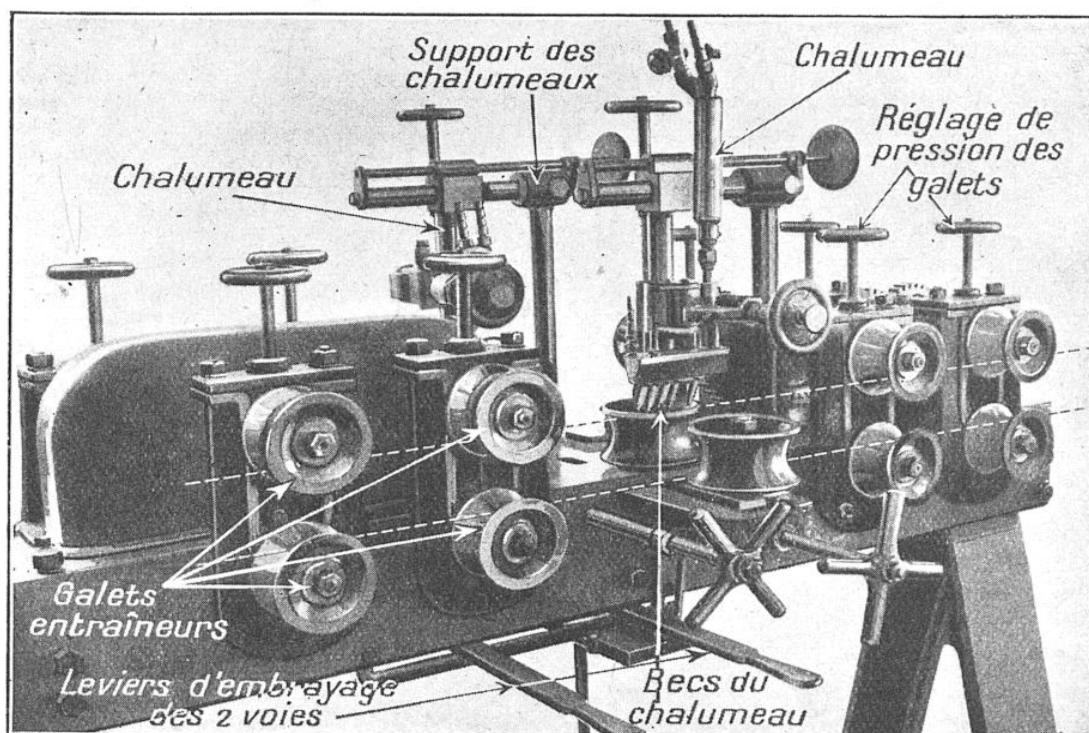
FIG. 23. — MACHINE A SOUDER LES TUBES, A DEUX VOIES, DE LA « S. A. F. »
