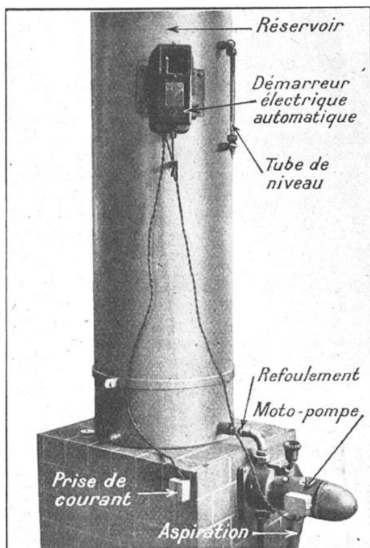
FIG. 18. — RÉSERVOIR « RENÉ VOLET » A DÉMARREUR AUTOMATIQUE
