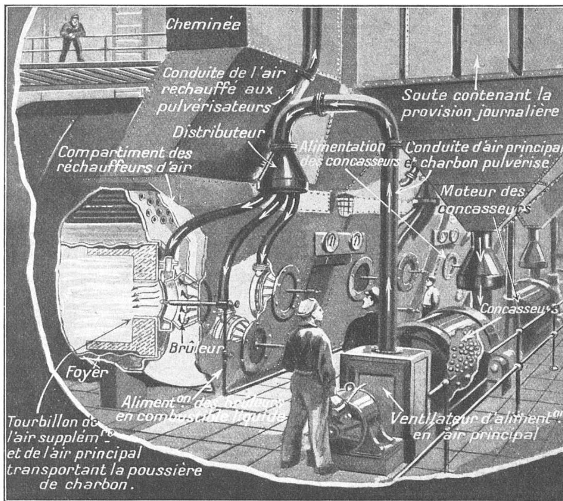
INSTALLATION DU « MERCER » POUR LA CHAUFFE AU CHARBON PULVÉRISÉ
