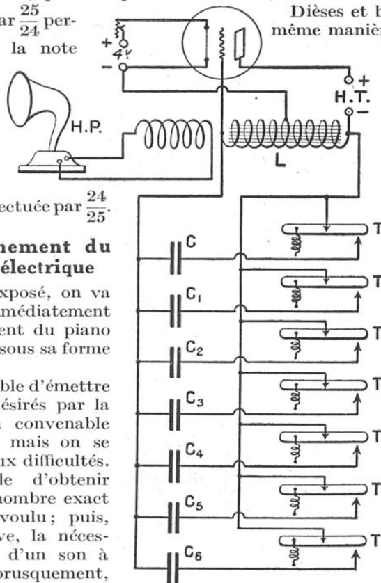
FIG. 3. — SCHÉMA DU PIANO RADIOÉLECTRIQUE
