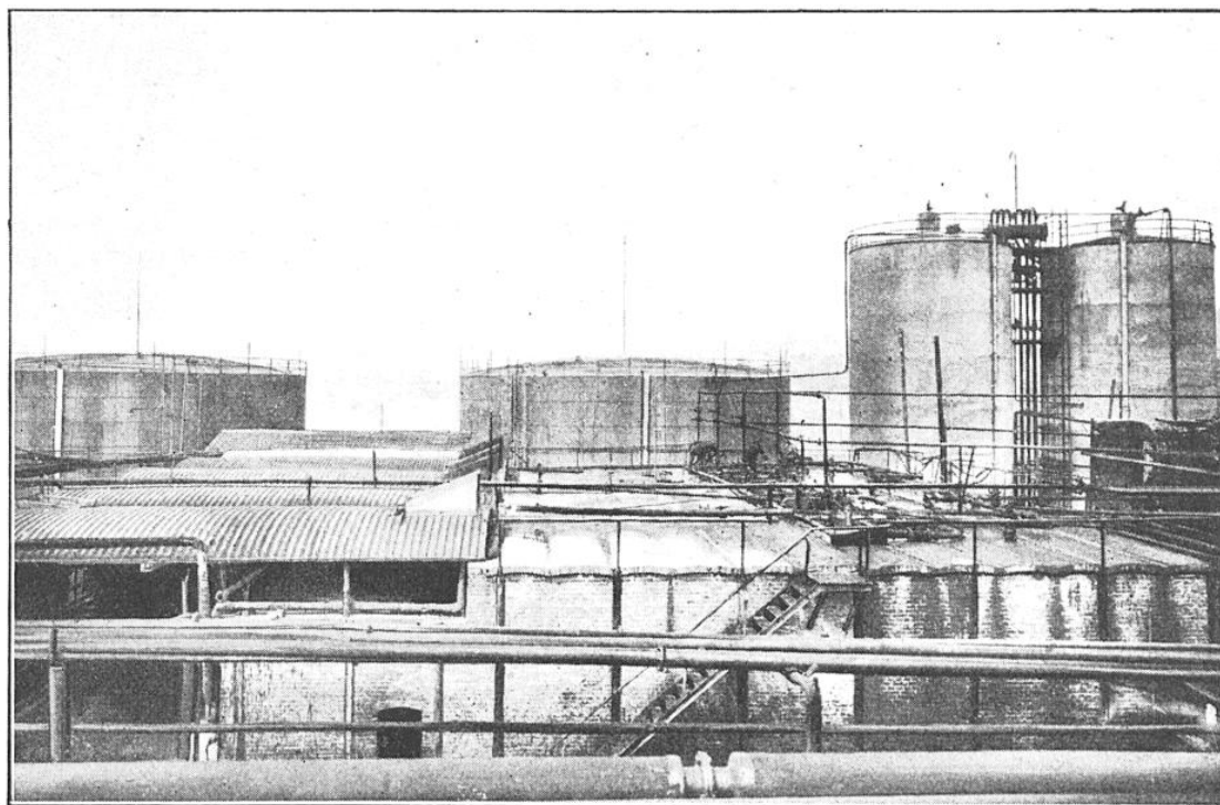
RÉSÉROIRS D'HUILE BRUTE ET CHAMBRES DE PREMIÈRE DISTILLATION DE PECHELBRONN
