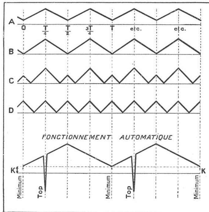
FIG. 4. — LE RYTHME DES BATTEMENTS PERÇUS PAR LE NAVIRE EN MARCHÉ (SUIVANT LE TRAJET PORTÉ DANS LA FIGURE PRÉCÉDENTE)
