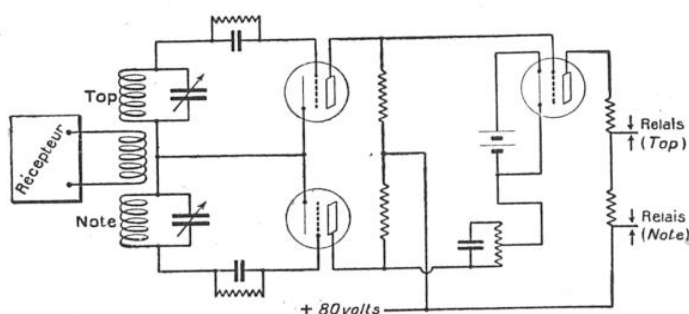
FIG. 5. — LA RÉCEPTION DIFFÉRENTIELLE A RELAIS
