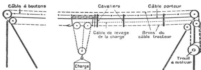
FIG. 2. — SCHÉMA D'UN TRANSPORTEUR PAR CÂBLE, TYPE « BLONDIN »
