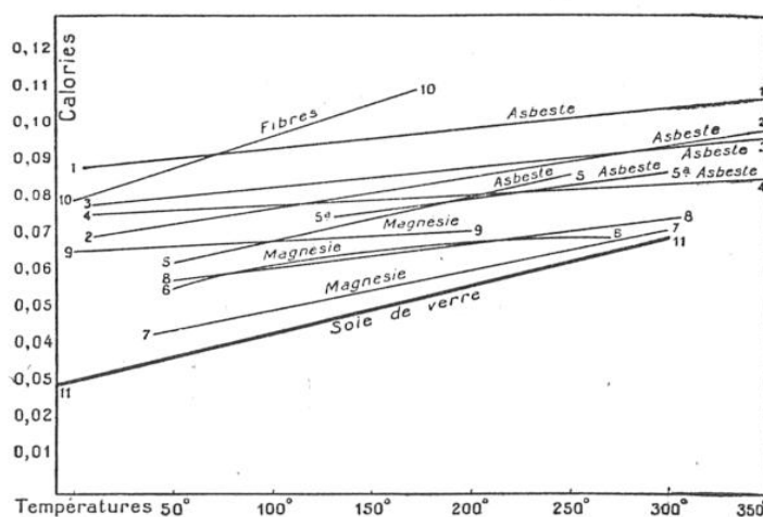
FIG. 5. — GRAPHIQUE COMPARATIF DES POUVOIRS ÉMISSIFS DES PRINCIPAUX CALORIFUGES
