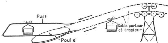
FIG. 5. - SYSTÈME DE TRANSPORTEUR PAR « MONOCABLE » Station terminale avec rails suspendus et pylône muni de poulies, sur lesquelles roule le monocable, emportant ses wagonnets.
