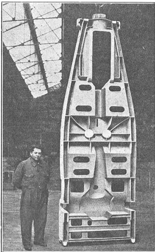
CHASSIS MONOBLOC EN ALPAX (1 M 40 SUR 4 M, 130 KG). (FOND. ET FORGES DE CRANS)
