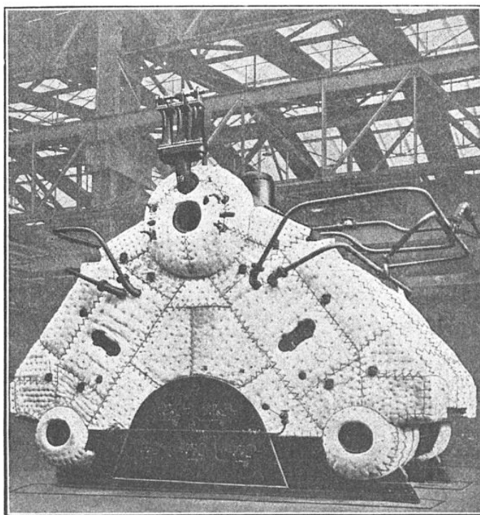
FIG. 7. — UNE CHAUDIÈRE MARINE DU PAQUEBOT « S. S. CAP. ARCONA » (27.000 TONNES), COMPLÈTEMENT CALORIFUGÉE A LA SOIE DE VERRE
