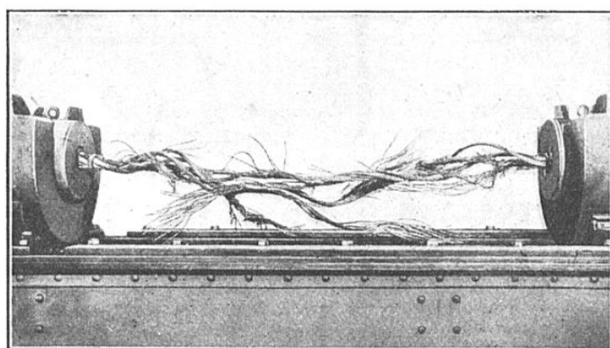
FIG. 8. — RUPTURE D'UN CÂBLE SUR LA MACHINE D'ESSAI REPRÉSENTÉE SUR LA FIGURE 7 CI-DESSUS
