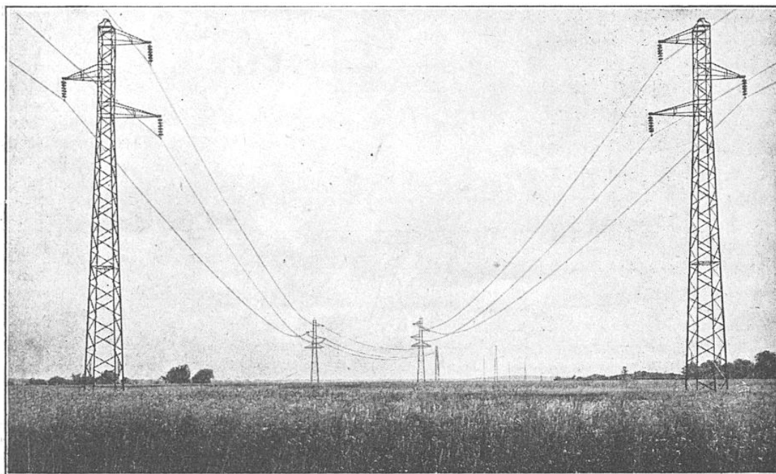
ÉLECTRIFICATION DU CHEMIN DE FER DE PARIS A ORLÉANS. LIGNE A 90.000 VOLTS PARIS-ÉGUZON EN ALUMINIUM-ACIER (ALUMINIUM FRANÇAIS)
