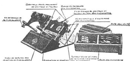
Stéréoscope de démonstration et d'entraînement.
