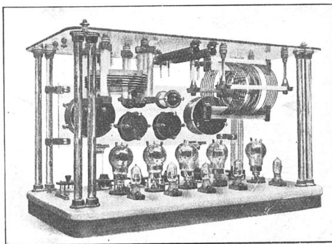
FIG. 7. — L'APPAREIL D'ÉMISSION UTILISÉ PAR LE COMMANDANT AICARDI
