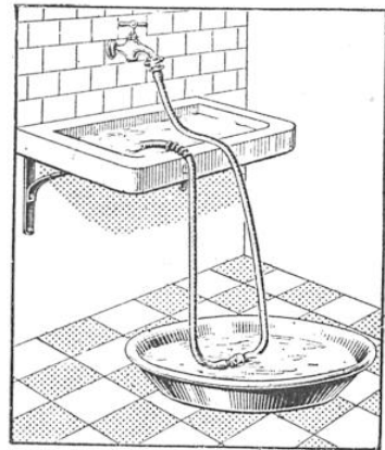
LE MÊME APPAREIL PLACÉ DANS LE TUB ASSURE AUTOMATIQUEMENT LA VIDANGE DE CELUI-CI DANS L'ÉVIER
