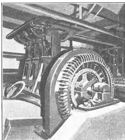
FIG. 7. — COMPRESSEUR CENTRIFUGE SERVANT AU CONDITIONNEMENT DE L'AIR DANS LES MAGASINS J. L. HUDSON (DETROIT)
