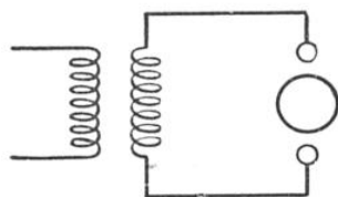
EXCITATEUR DE LODGE POUR ONDES DE QUELQUES CENTIMÈTRES
