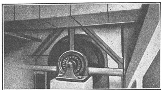
FIG. 1. — VENTILATEUR PRINCIPAL D'UNE UNITÉ DE CONDITIONNEMENT DE L'AIR DE L'UNION TRUST BUILDING
