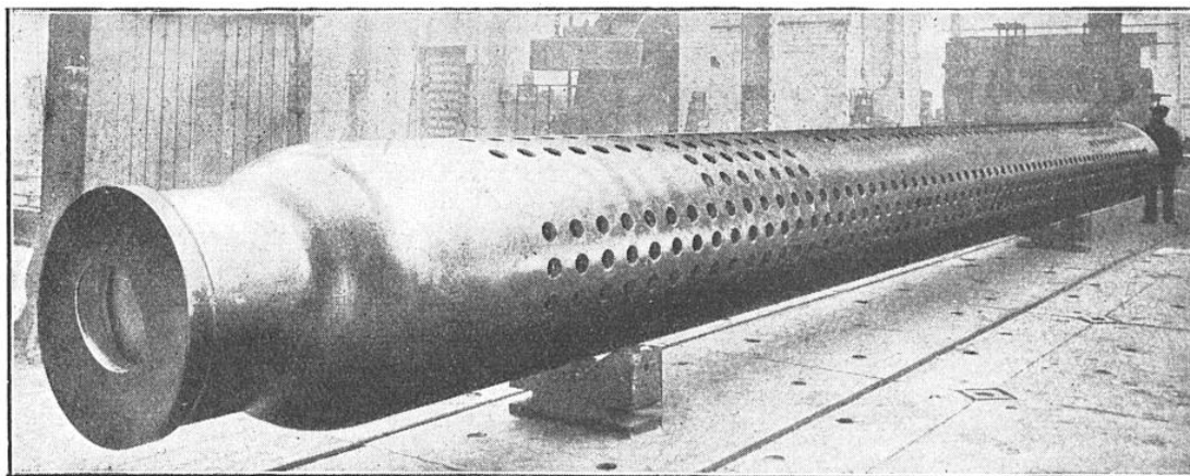
LE CORPS DE CHAUDIÈRE TERMINÉ PEUT RÉSISTER A UNE PRESSION DE 60 KG PAR CM 2 Les cercles noirs de cette photo représentent les trous où viennent s'adapter les tubes de vaporisation.
