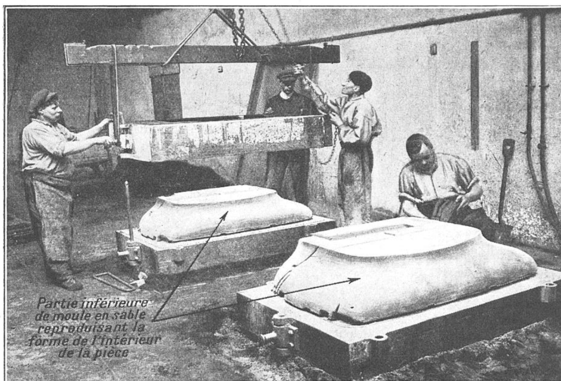
UNE OPÉRATION DU MOULAGE A LA MACHINE D'UN TABLIER DE CAMION AUTOMOBILE, DANS UNE FONDERIE AU SABLE
