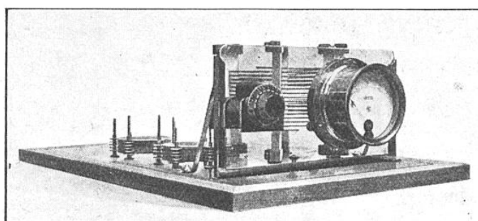
FIG. 8. — CONDENSATEUR TOURNANT, DESTINÉ A FAIRE VARIER LE DÉPHASAGE DES ONDES ET, PAR CONSÉQUENT, LA POSITION DE LA LIGNE NODALE
