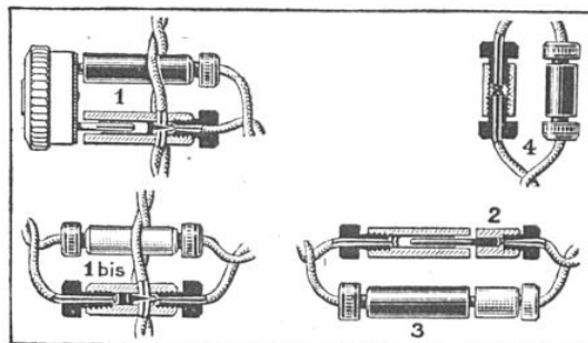
QUELQUES MODÈLES DE PRISES DE COURANT OU RACCORDS ÉLECTRIQUES À POSE INSTAN- TANÉE « RAYO »
