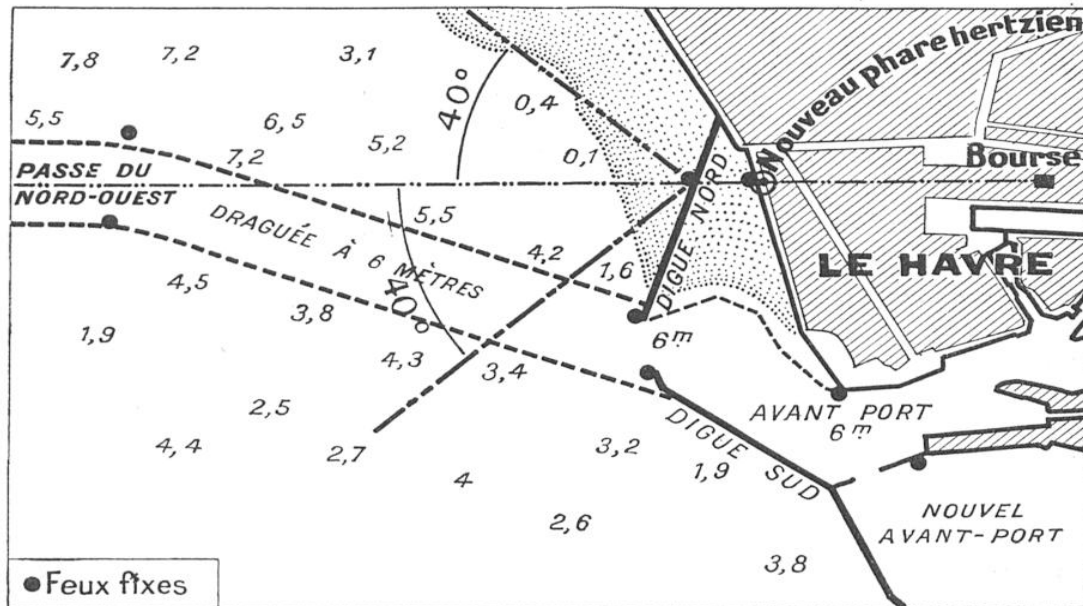
FIG. 1. — LA STATION D'ESSAI DES ALIGNEMENTS HERTZIENS DU COMMANDANT AICARDI, POUR FACILITER L'ENTRÉE DES NAVIRES DANS LE PORT DU HAVRE
