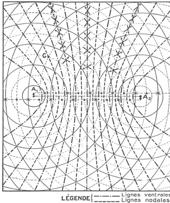
FIG. 2. - SCHÉMA MONTRANT LE MÉCANISME DES INTERFÉRENCES D'ONDES
