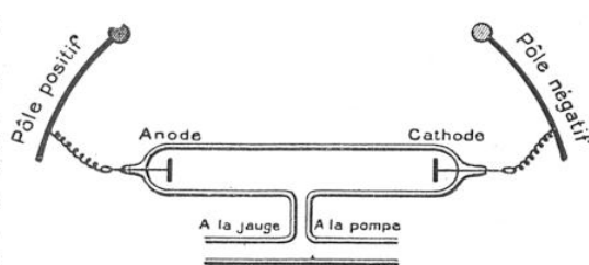
FIG. 1. — COMMENT ON ÉTUDIE LA LUMINESCENCE DES TUBES A VIDE
