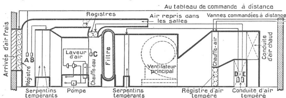
FIG. 4. — SCHÉMA D'UNE UNITÉ DE CONDITIONNEMENT DE L'AIR DES ÉTABLISSEMENTS DETROIT EDISON, A DETROIT
