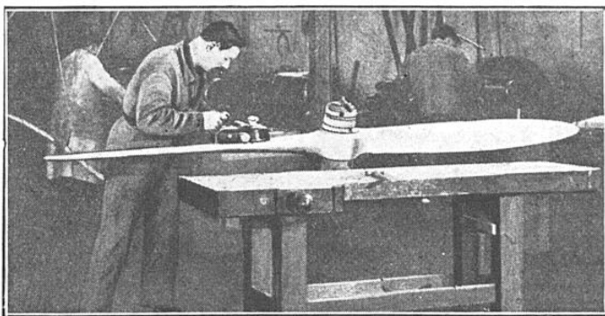
RABOTAGE FINAL D'UNE HÉLICE FORGÉE EN DURALUMIN (ALUMINIUM FRANÇAIS)
