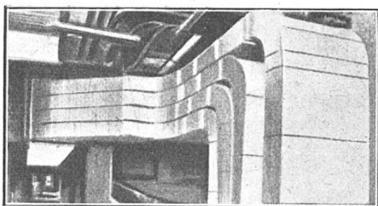
FIG. 5. — LES CONDUITES D'AIR CONDITIONNÉ, SITUÉES DANS LE SOUS-SOL DE L'IMMEUBLE DE L'UNION TRUST CO (DETROIT), SONT DISPOSÉES DE MANIÈRE A RÉDUIRE L'ENCOMBREMENT AU MINIMUM
