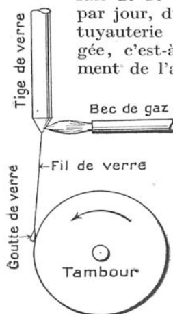
FIG. 1. — PRINCIPE DE LA PRÉPARATION DES FILS DE VERRE
