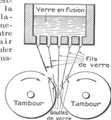
FIG. 2. — SCHÉMA DE LA PRÉPARATION INDUSTRIELLE DES FILS DE VERRE
