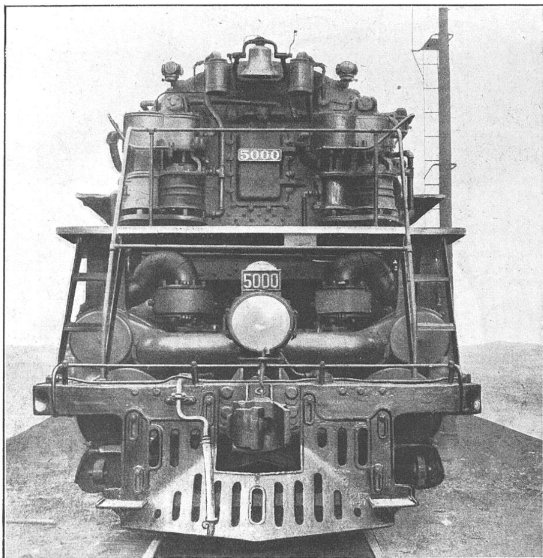
VUE AVANT DE LA LOCOMOTIVE DE 6.000 CH DU NORTHERN PACIFIC RAILWAY
