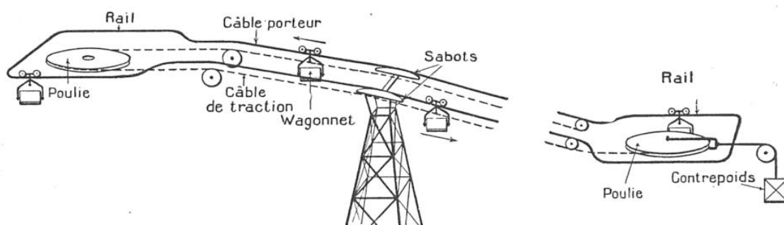
FIG. 3. — SCHÉMA D'UN TRANSPORTEUR PAR CABLE, TYPE « TRICÂBLE » CONTINU
