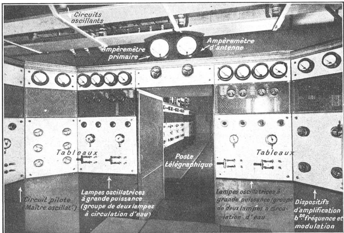
ENSEMBLE DU NOUVEAU POSTE RADIOTÉLÉPHONIQUE DE LA TOUR EIFFEL
