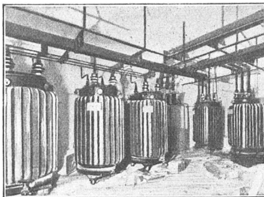
FIG. 9. — CHAMBRE DES TRANSFORMATEURS DANS LE SOUS-SOL D'UN BUILDING
