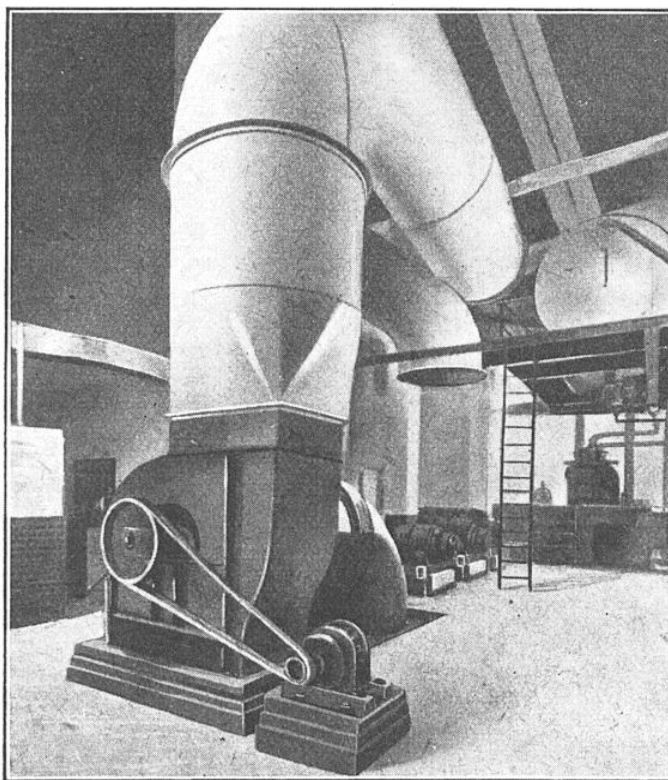
FIG. 6. — DISPOSITIF DE VENTILATION, PAR ASPIRATION, DES LIEUX PUBLICS, ESCALIERS, COULOIRS, TOILETTES, ETC., DANS UN DES PLUS HAUTS GRATTE-CIEL AMÉRICAINS DE DETROIT
