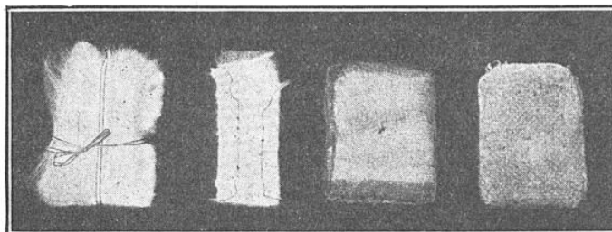
FIG. 6. — LES DIVERSES FORMES DE LA SOIE DE VERRE De gauche à droite : bourrage, feutre et matelas de soie de verre.
