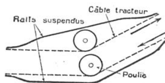
FIG. 4. — STATION D'ANGLE D'UN TRICÂBLE, AVEC DÉCROCHAGE DES WAGONNETS, QUI ROULENT SUR DES RAILS SUSPENDUS
