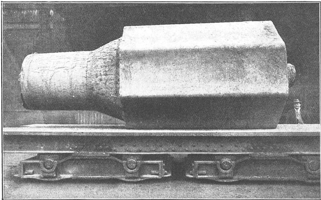
LE BLOC D'ACIER QUI VA ÊTRE PERFORÉ, A LA MANIÈRE D'UN CANON, AVANT D'ÊTRE TRANSFORMÉ EN CORPS DE CHAUDIÈRE
