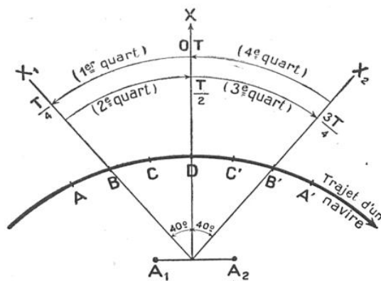
FIG. 3. — DISPOSITIF SCHÉMATIQUE DES RADIOALIGNEMENTS FIGURANT SUR LA CARTE (FIG. 1)
