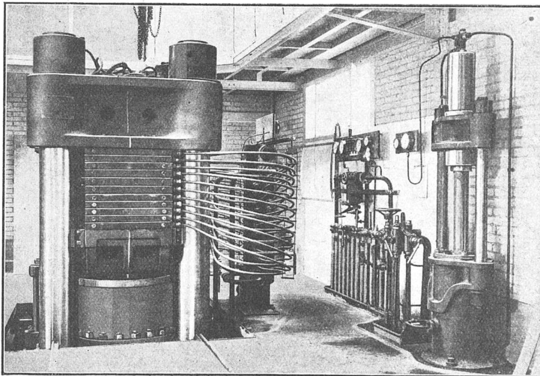
FIG. 4. — DANS CETTE « PRESSE A BLOCS », CHAUFFÉE PAR UNE CIRCULATION DE VAPEUR, LES LAMES DE NACRE ARTIFICIELLE SONT SOUDÉES ENSEMBLE POUR FORMER DES BLOCS QUI SONT ENSUITE DÉBITÉS EN FEUILLES
