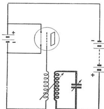
OSCILLATEUR A LAMPE
