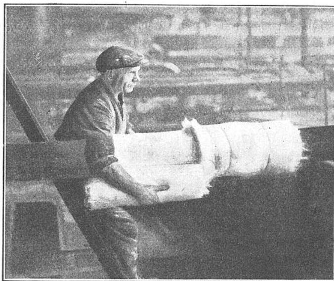
FIG. 9. — ON POSE LA SOIE DE VERRE SUR UN TUYAU EN ENROULANT SIMPLEMENT AUTOUR DE LUI UN OU PLUSIEURS MATELAS DE CE CALORIFUGE
