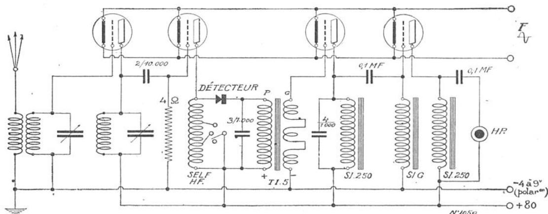
MONTAGE D'UN RÉCEPTEUR AVEC TRANSFORMATEUR « SOLOR TI. 5 », SELF DE LIAISON « SI. 250 » ET SELF DE POLARISATION DE GRILLE « SI. G »
