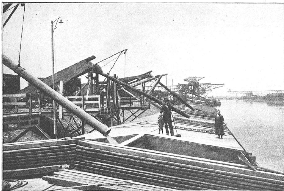
L'EMBARQUEMENT DES POTASSES D'ALSACE SUR LES CHALANDS QUI L'AMÈNENT EN GRANDE PARTIE AU PORT D'ANVERS (1) SE FAIT AUTOMATIQUEMENT AU MOYEN DE TRANSPORTEURS ET DE TUYAUX QUI RÉPARTISSENT LA POTASSE DANS LA CALE
