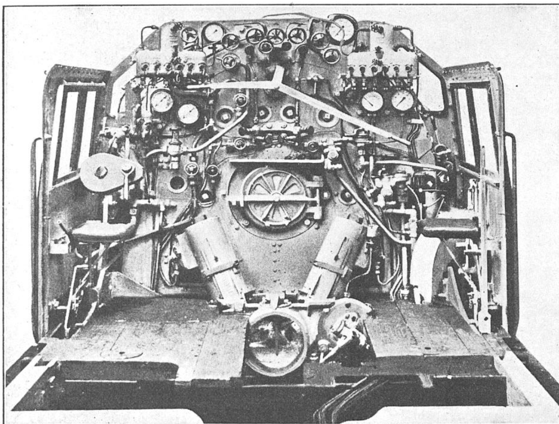
L'ARRIÈRE DE LA LOCOMOTIVE GARRATT, MONTRANT LA COMPLEXITÉ DES COMMANDES MISES A LA DISPOSITION DU MÉCANICIEN
