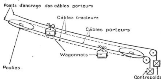
FIG. 1. — SCHÉMA D'UN TRANSPORTEUR PAR CÂBLE TYPE « VA-ET-VIENT »
