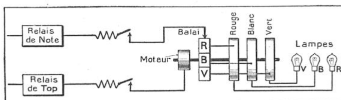
FIG. 6. — L'APPAREIL AUTOMATIQUE A LAMPES
