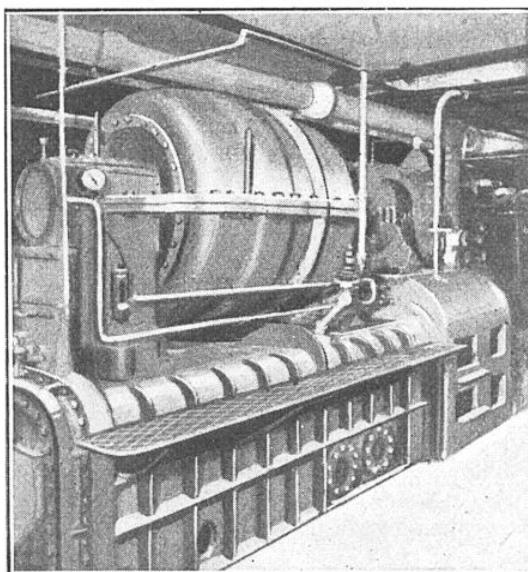
FIG. 3. — COMPRESSEUR A GAZ CARBONIQUE UTILISÉ POUR LE CONDITIONNEMENT DE L'AIR DANS L'UNION TRUST BUILDING
