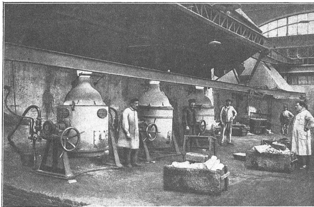
BATTERIE DE FOURS DE FUSION BASCULANTS CHAUFFÉS A L'HUILE LOURDE
