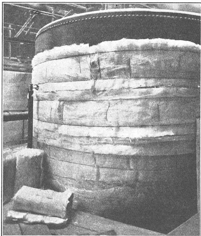
FIG. 8. — UN RÉSERVOIR A HUILE CALORIFUGÉ PAR UN ÉPAIS MATELAS DE SOIE DE VERRE
