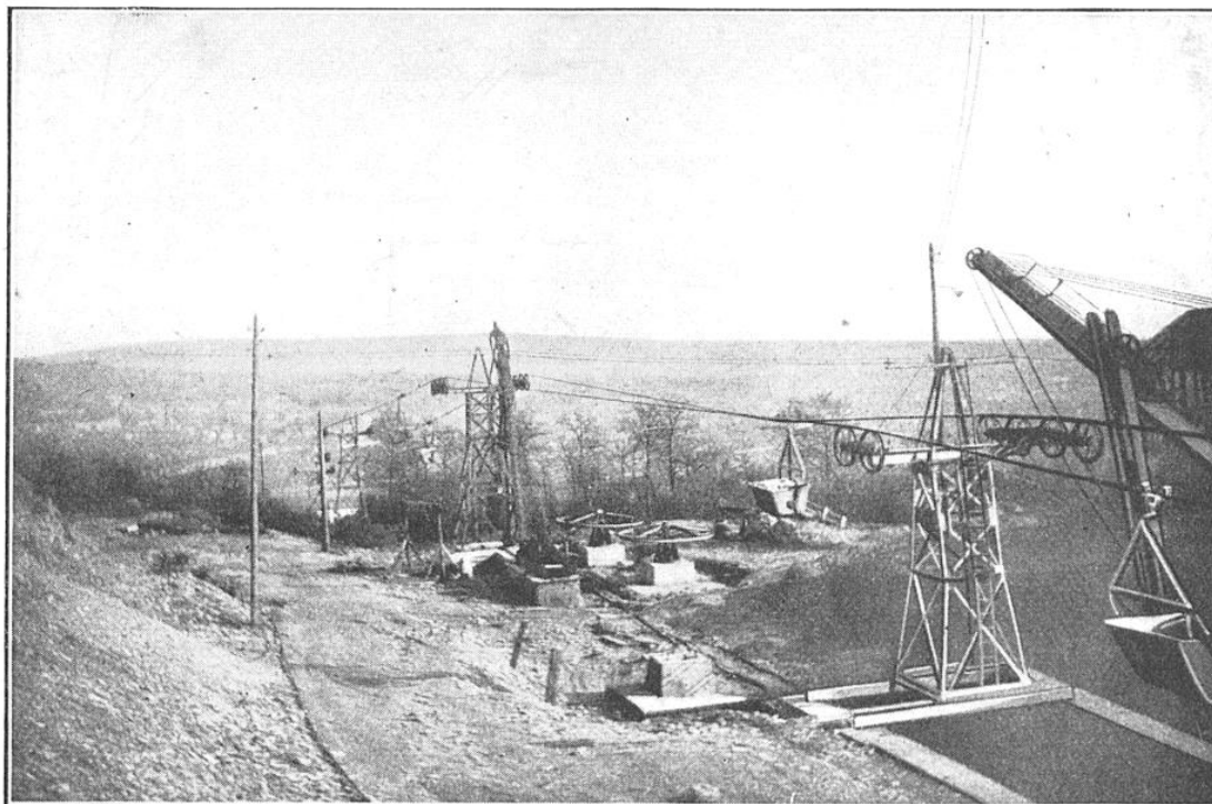
FIG. 10. — DÉPART DE LA STATION DE CHARGEMENT DU « MONOCABLE » DE MAXÉVILLE-DOMBASLE ET DISPOSITIF DE TENSION DU CÂBLE
