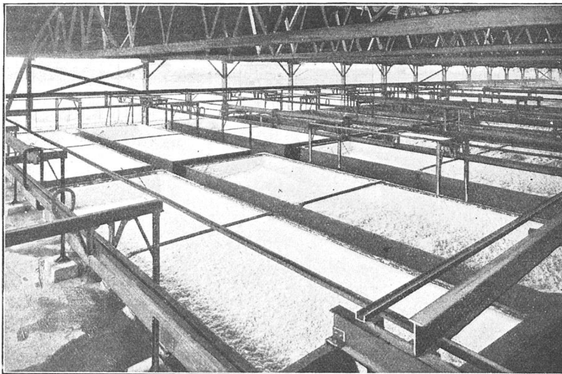
BASSINS DE CRISTALLISATION OU LE CHLORURE DE POTASSIUM SE DÉPOSE
