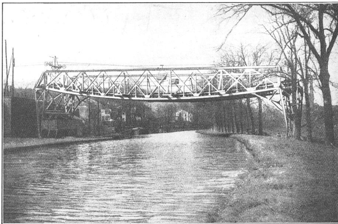
FIG. 11. — PONT-ABRI SUR LE CANAL DE LA MARNE AU RHIN
