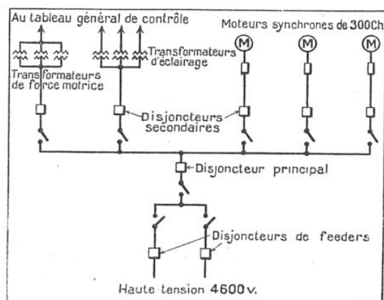
FIG. 8. — SCHÉMA DE L'INSTALLATION ÉLECTRIQUE À HAUTE TENSION DE L'UNION TRUST BUILDING (DETROIT)
