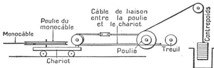
FIG. 6. — DISPOSITIF DE TENSION DU « MONOCABLE » Le treuil permet de déplacer, selon les besoins, le chariot portant la poulie du monocable, tout en laissant sa tension réglée automatiquement par le contrepoids.
