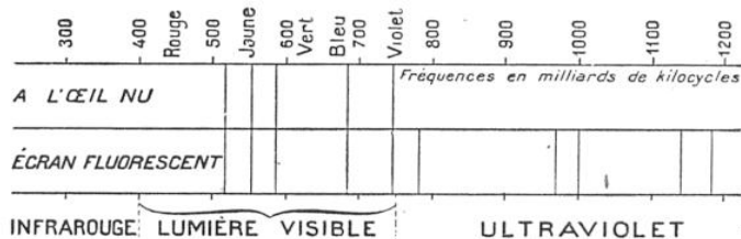
FIG. 14. — RADIATIONS ÉMISES PAR LA VAPEUR DE MERCURE
