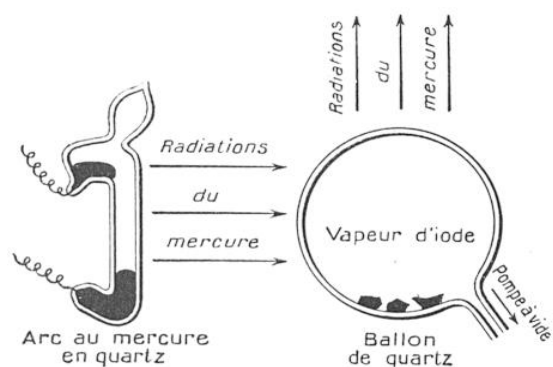
FIG. 16. - EN QUOI CONSISTE L'EFFET WOOD
