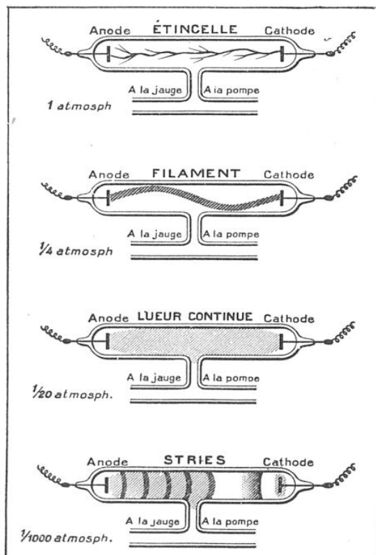
FIG. 2, 3, 4, 5. — DIFFÉRENTS ASPECTS DE LA DÉCHARGE ÉLECTRIQUE
