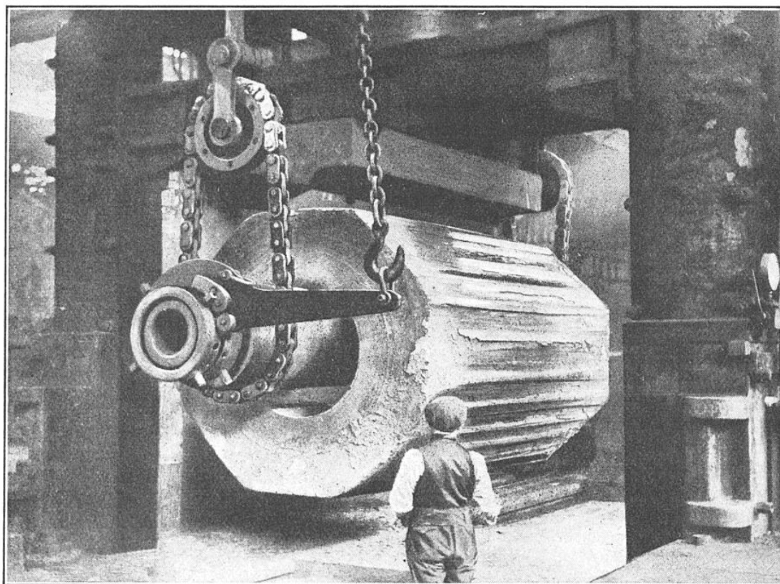
LE BLOC D'ACIER PERFORÉ, APRÈS AVOIR ÉTÉ CHAUFFÉ, EST FORGÉ, DE MANIÈRE À ÊTRE ÉTIRÉ POUR FORMER LE CORPS DE LA CHAUDIÈRE
