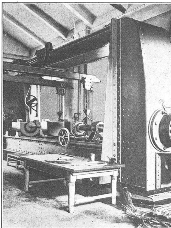
FIG. 7. — ENSEMBLE DE LA MACHINE DE 250 TONNES DES LABORATOIRES DES MINES DE LA SARRE, DISPOSÉE POUR L'ESSAI DE TRACTION D'UN CÂBLE
