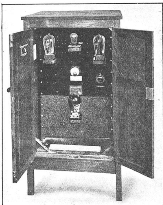
FIG. 2. — INTÉRIEUR DE L'ARMOIRE-AMPLIFICATEUR, LES PORTES ÉTANT OUVERTES
