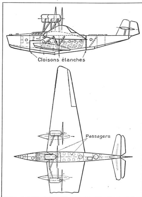
ÉLÉVATION ET VUE EN PLAN DU « ROHRBACH-ROMAR » DE 19,5 TONNES
