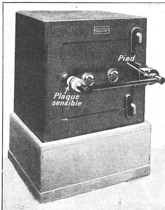
APPAREIL DE PROTECTION CONTRE L'INCENDIE DE COFFRES-FORTS ET DE CHAMBRES FORTES
