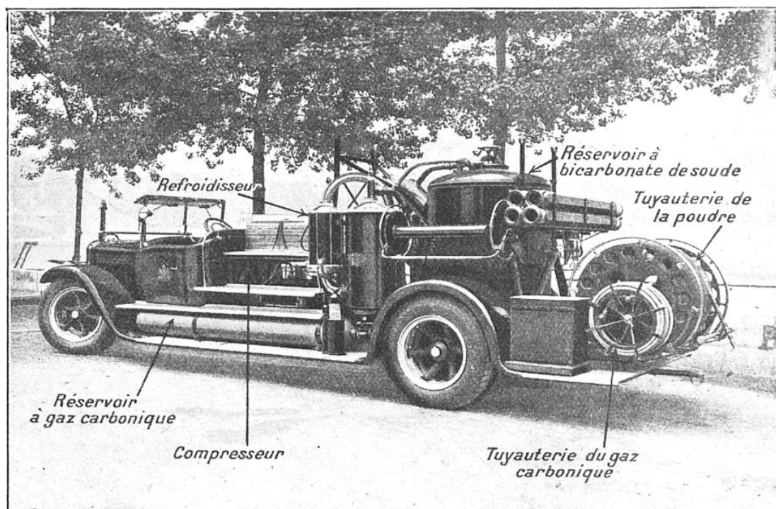
VUE D'ENSEMBLE D'UNE MACHINE A PROJETER UNE POUDRE EXTINGUANTE
