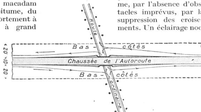
FIG. 3. — COMMENT L'AUTOROUTE SE RACCORDERA AVEC UNE ROUTE ORDINAIRE QU'ELLE FRANCHIT SUR UN PONT. On voit qu'une automobile peut entrer en vitesse dans les deux sens sur l'autoroute et en sortir sans aucune manœuvre compliquée pour passer sur un chemin ordinaire.
