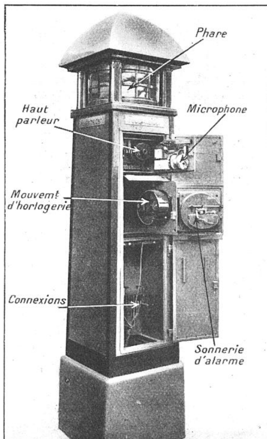
AVERTISSEUR PUBLIC « SIEMENS-FRANCE », MODÈLE SUR COLONNE
