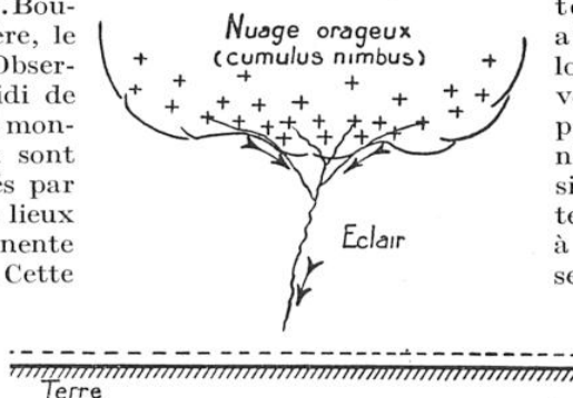
FIG. 1. — SCHÉMA MONTRANT LE MÉCANISME DE LA DÉCHARGE DE LA FOUDRE
