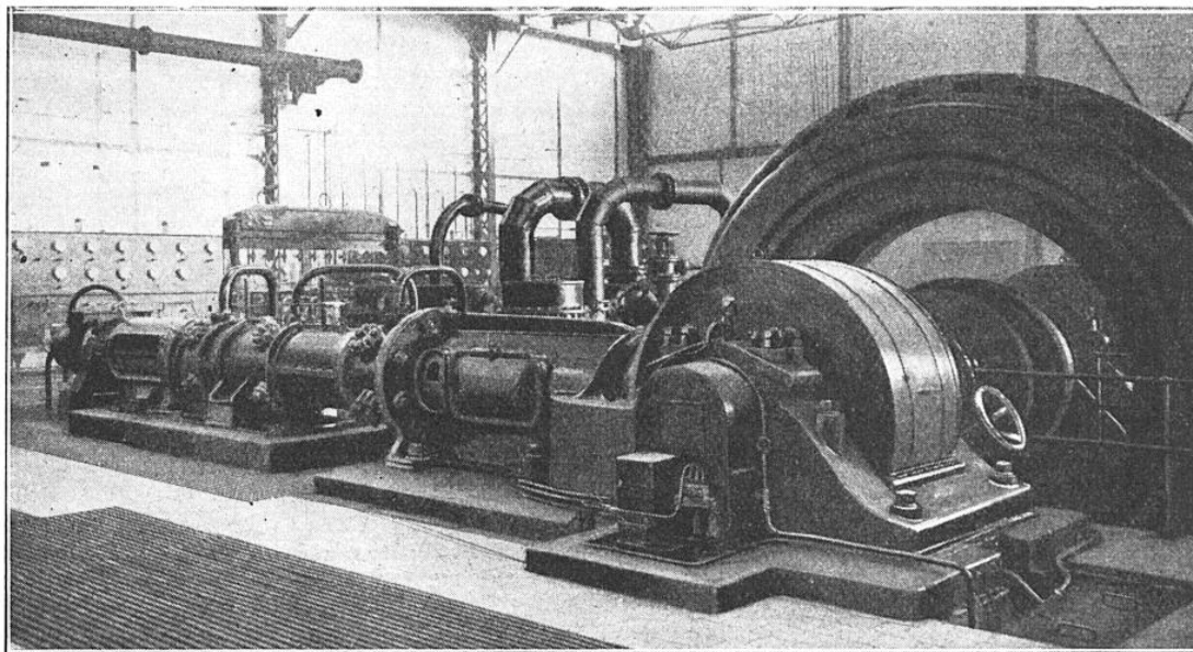
HYPERCOMPRESSEUR DE L'USINE DE WAZIERS, COMPRIMANT 3.300 MÈTRES CUBES À L'HEURE DE MÉLANGE D'AZOTE ET D'HYDROGÈNE À 1.000 ATMOSPHÈRES, POUR LA FABRICATION D'AMMONIAQUE SYNTHÉTIQUE PAR LE PROCÉDÉ GEORGES CLAUDE
