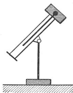
FIG. 4. — SCHÉMA D'UN PYRRHÉLIOMÈTRE SERVANT A MESURER LE RAYONNEMENT SOLAIRE
