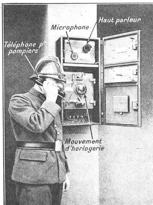
AVERTISSEUR PUBLIC « SIEMENS-FRANCE », MODÈLE MURAL
