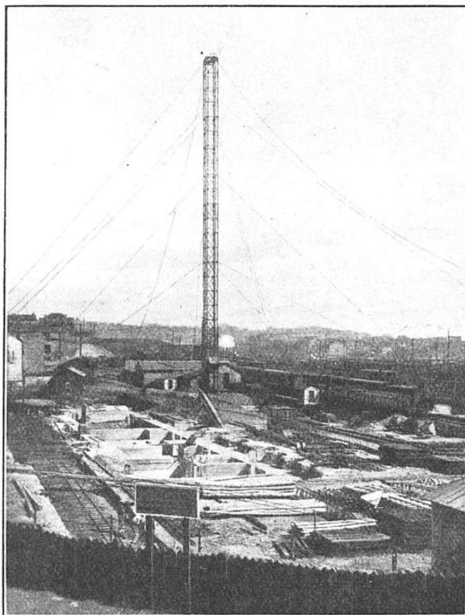
TOUR A BÉTON DE 60 MÈTRES DE HAUTEUR TOTALE EN COURS DE MONTAGE
