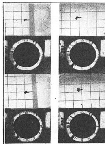
UNE PARCELLE DU FILM OBTENU, MONTRANT QUATRE POSITIONS DIFFÉRENTES D'UN AVION AVEC, AU-DESSOUS, LE CADRAN DU CHRONOMÈTRE INDICANT LES TEMPS.
