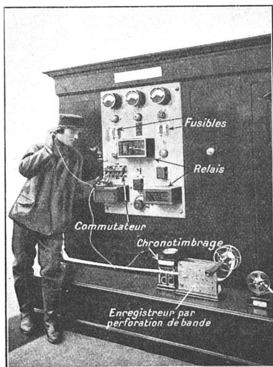
BUREAU CENTRAL DE POMPIERS DE LA « GAMEWELL FIRE ALARM »
