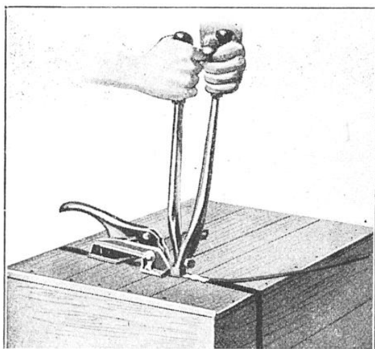
COMMENT ON SERTIT LE « SIGNODE » POUR FIXER LA BANDE D'ACIER
