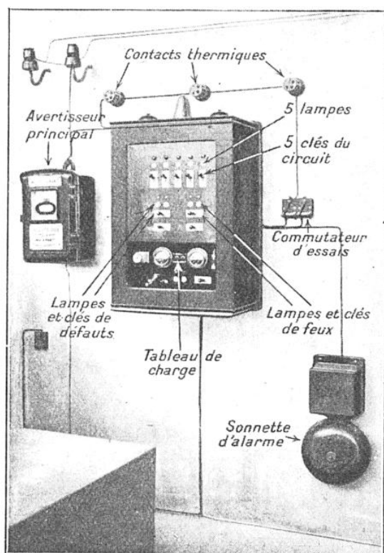
BUREAU CENTRAL DE SECOURS, SYSTÈME « ERICSSON »
