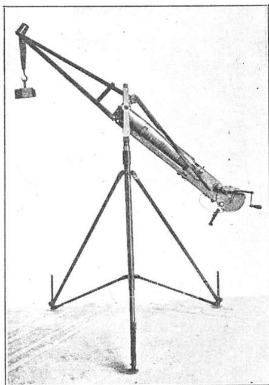
LA CINÉMITRAILLEUSE « H. M. P. »
