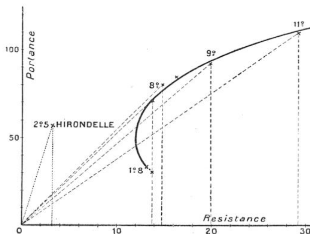
EXEMPLE D'UNE COURBE « POLAIRE » RELATIVE A UN AÉROPLANE :
