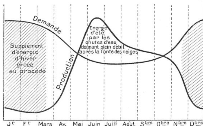
FIG. 4. — GRAPHIQUE MONTRANT QUELLE DISPROPORTION SÉPARE, EN TOUT MOIS DE L'ANNÉE, LA DEMANDE ET LA PRODUCTION DE L'ÉLECTRICITÉ DANS LE CANADA SEPTENTRIONAL.
