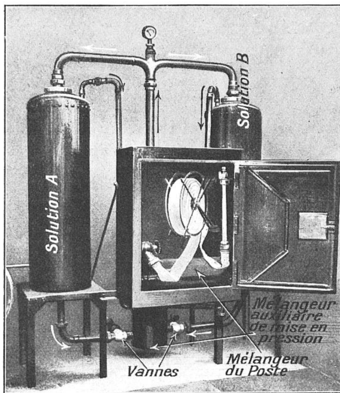
APPAREIL PRODUCTEUR DE MOUSSE SOUS PRESSION « PHILLIPS ET PAIN »
