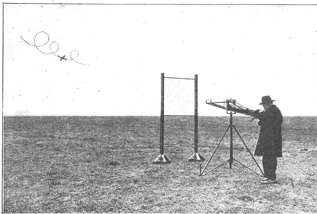
LA CINÉMITRAILLEUSE « H. M. P. » EN ACTION
