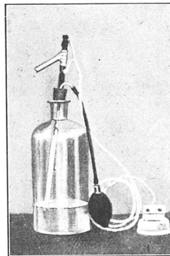
IL SUFFIT D'APPUYER SUR LA POIRE EN CAOUTCHOUC DE CET APPAREIL POUR OBTENIR UN ÉCOULEMENT D'EAU CHAUDE PAR L'AJUTAGE SUPÉRIEUR
