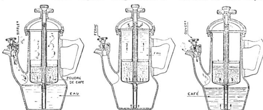
TROIS PHASES DE LA PRÉPARATION DU CAFÉ AVEC LE « PERCO-THERMOS »
