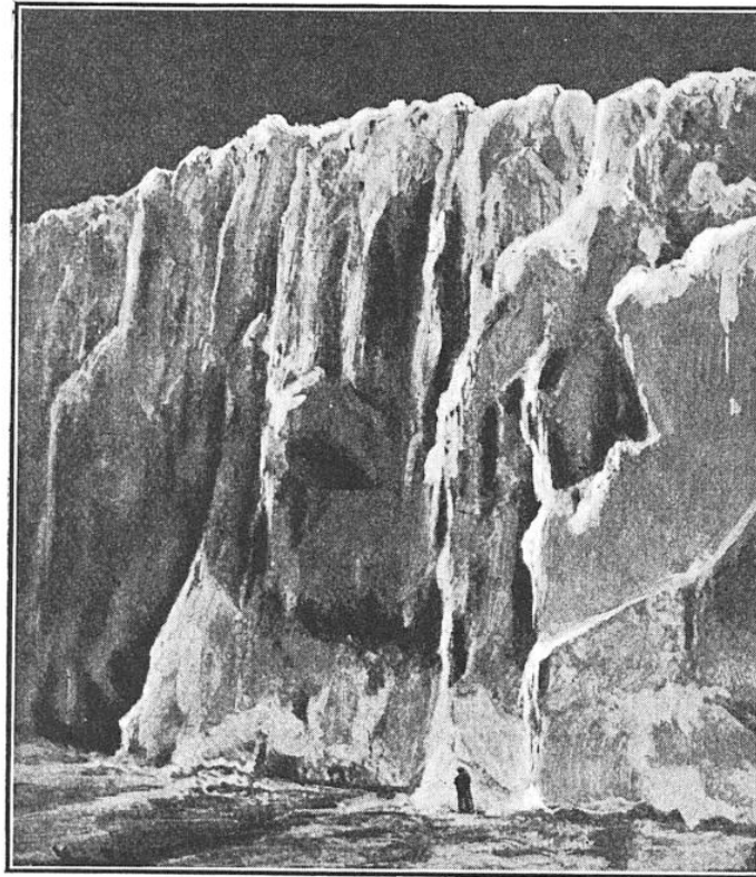
FIG. 5. — LE RAYONNEMENT SOLAIRE PERMETTRAIT DE FONDRE ANNUELLEMENT CETTE FALAISE DE GLACE HAUTE DE 120 MÈTRES
