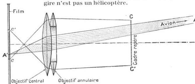
L'OBJECTIF DE LA CINÉMITRAILLEUSE
