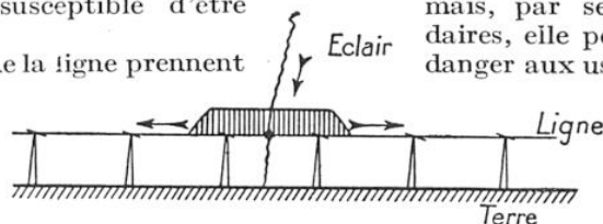
FIG. 2. — LA Foudre tombant sur une ligne électrique provoque la formation de deux ondes se propageant de part et d'autre du point influencé
