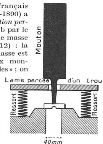
FIG. 14. — LE CHOC DONNE UNE MESURE DE LA FRAGILITÉ
