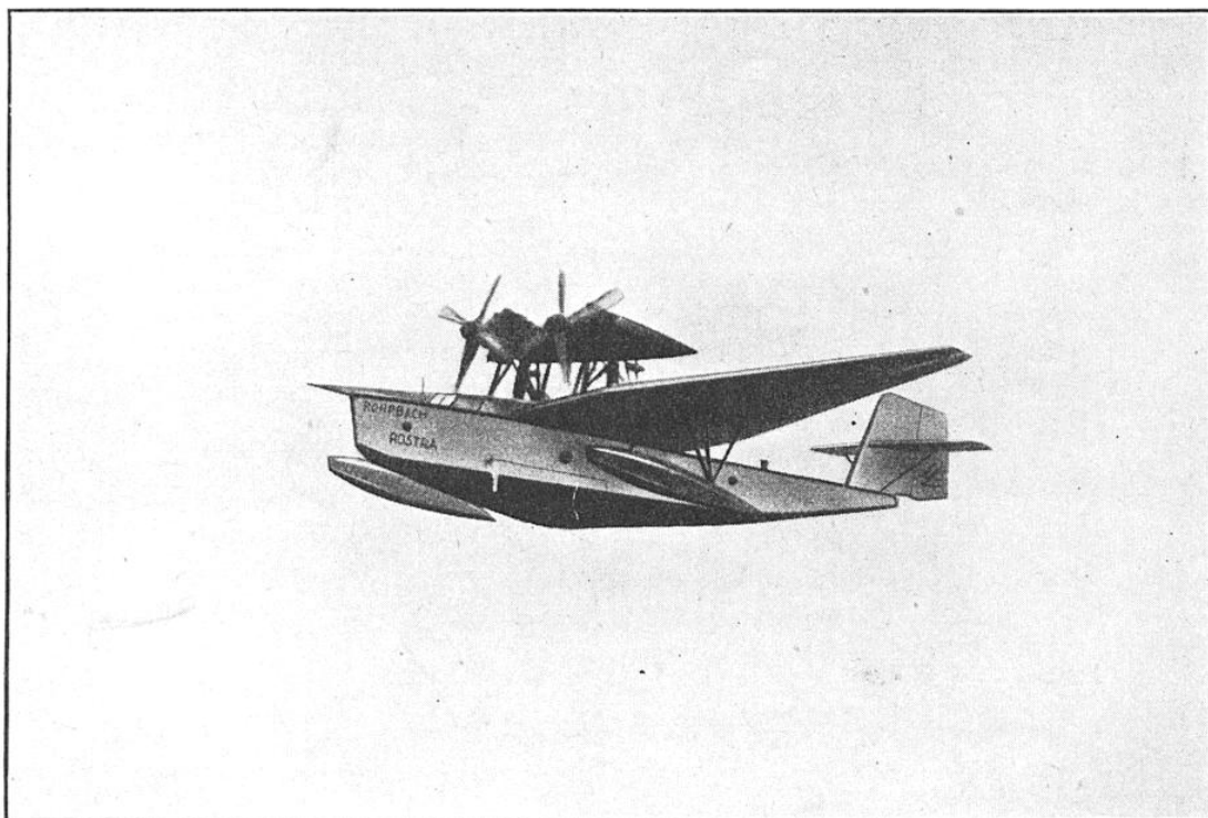
LE « ROHRBACH-ROSTRA » EN VOL
