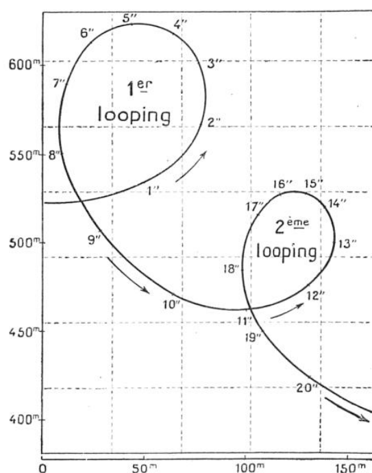
UNE TRAJECTOIRE D'AVION RECONSTITUÉE DE SECONDE EN SECONDE
