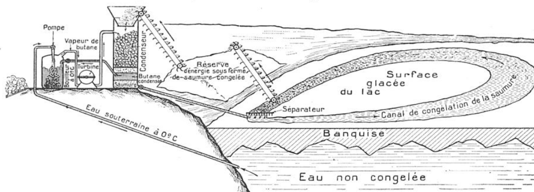
FIG. 1. — SCHÉMA DU FONCTIONNEMENT GÉNÉRAL DE L'USINE POLAIRE
