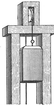
FIG. 15. — MOUTON POUR « BATTRE » LES PIEUX
