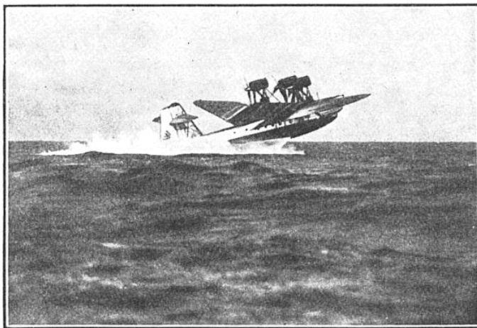
LE « ROHRBACH-ROMAR » AU COURS DES ESSAIS DANS LA BAIE DE TRAVEMUNDE
