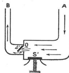
LE BÉLIER HYDRAULIQUE EST UNE APPLICATION DU CHOC
