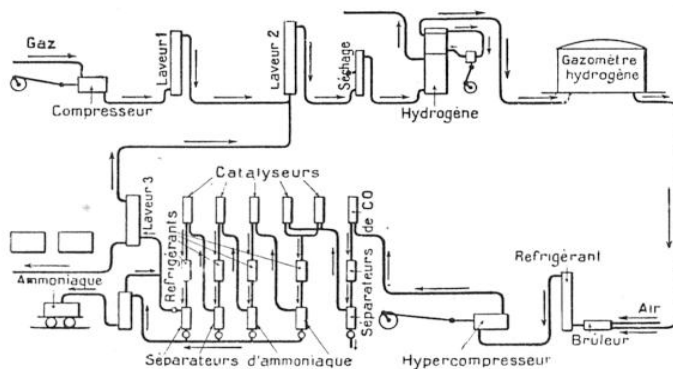
SCHÉMA DE FABRICATION DE L'AMMONIAQUE SYNTHÉTIQUE, A PARTIR DU GAZ DE FOURS A COKE, PAR LE PROCÉDÉ GEORGES CLAUDE
