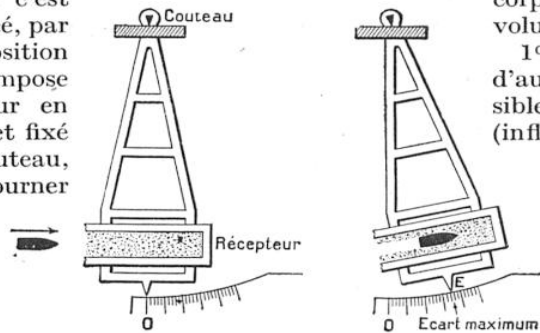
DEUXIÈME EXEMPLE DE CHOC : LE PENDULE BALISTIQUE
