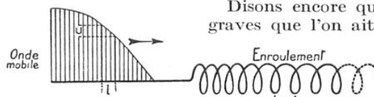
FIG. 3. — SCHÉMA MONTRANT L'ACCROISSEMENT DE LA TENSION ENTRE SPIRES DANS UN ENROULEMENT AU PASSAGE D'UNE ONDE
