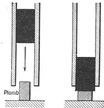
FIG. 12 ET 13 UN EXEMPLE DE CHOC MOU : L'ÉCRASEMENT DU PLOMB
