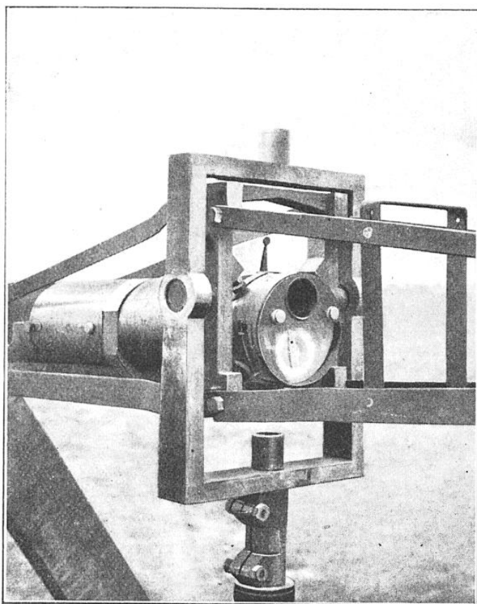
L'OBJECTIF DE LA CINÉMITRAILLEUSE SUR SON PIVOT A LA CARDAN
