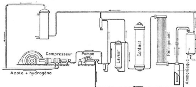
SCHEMA DE FABRICATION DE L'AMMONIAQUE SYNTHÉTIQUE PAR LE PROCÉDÉ CASALE
