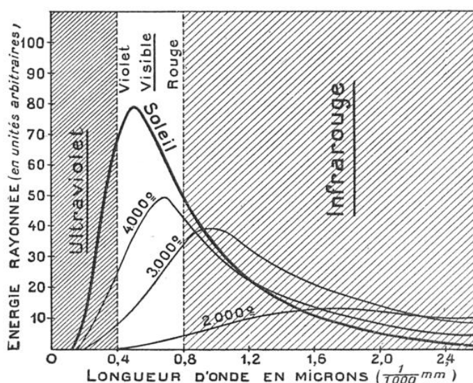
FIG. 3. — LA COMPARAISON ENTRE LE RAYONNEMENT SOLAIRE ET CELUI D'AUTRES SOURCES A PERMIS D'ÉVALUER A 6.500 DEGRÉS LA TEMPÉRATURE DE LA PHOTOSPHÈRE. Pour comparer à la même échelle verticale ces différentes courbes, il faut diviser les ordonnées de la courbe correspondant à 4.000° C par 5, celles de la courbe de 3.000° C par 17, celles de la courbe de 2.000° C par 33. De sorte que les courbes qui ont l'air de se couper (car les échelles ne sont pas les mêmes pour toutes) ne se coupent jamais en aucun de leurs points. Les échelles choisies sont nécessaires pour permettre une représentation commode sur le dessin.
