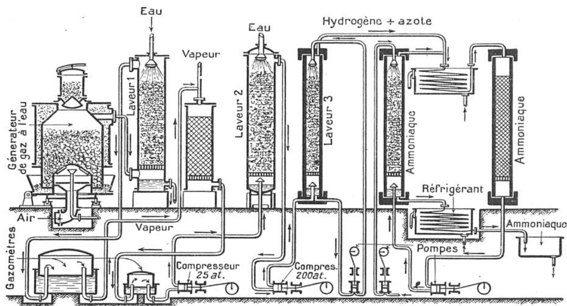
SCHEMA DE FABRICATION DE L'AMMONIAQUE SYNTHÉTIQUE PAR LE PROCÉDÉ HABER-BOSCH
