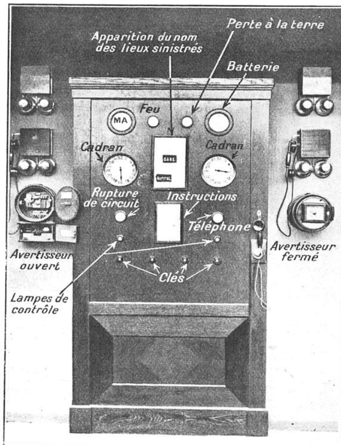
POSTE CENTRAL « SIEMENS-FRANCE », DESTINÉ AUX AGGLOMÉRATIONS D'IMPORTANCE MOYENNE
