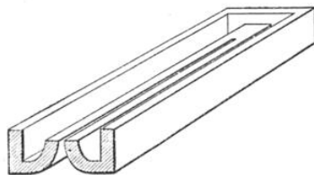
FIG. 9. — COUPE TRANSVERSALE ET VUE PERSPECTIVE DE LA « DÉBITEUSE » (PROCÉDÉ FOURCAULT)
