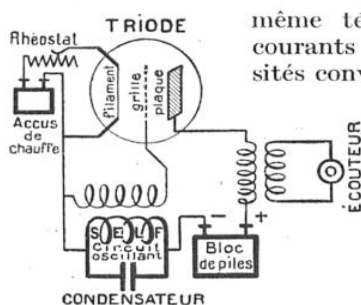
FIG. 13. — UN OSCILLATEUR A FRÉQUENCE AUDIBLE
