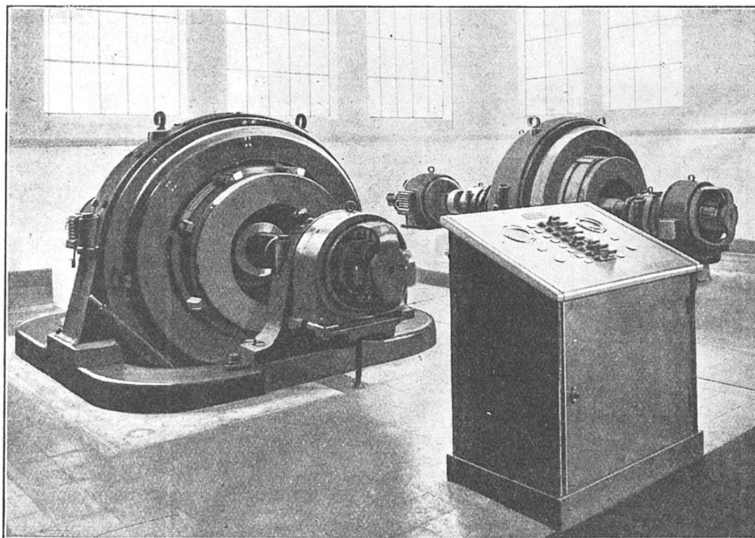
VUE INTÉRIEURE DE LA SOUS-STATION DU HOURAT (CHEMINS DE FER DU MIDI)
