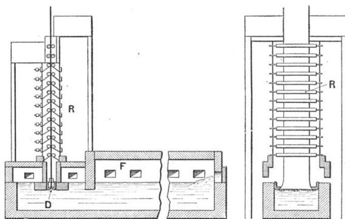
FIG. 12. — COUPES LONGITUDINALE ET TRANSVERSALE DU Puits d'étirage à rouleaux de la machine UTILISÉE DANS LE PROCÉDÉ FOURCAULT
