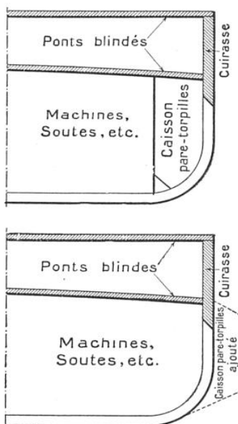
INFLUENCE DU SOUS-MARIN SUR LA PROTECTION DES GROS BATIMENTS
