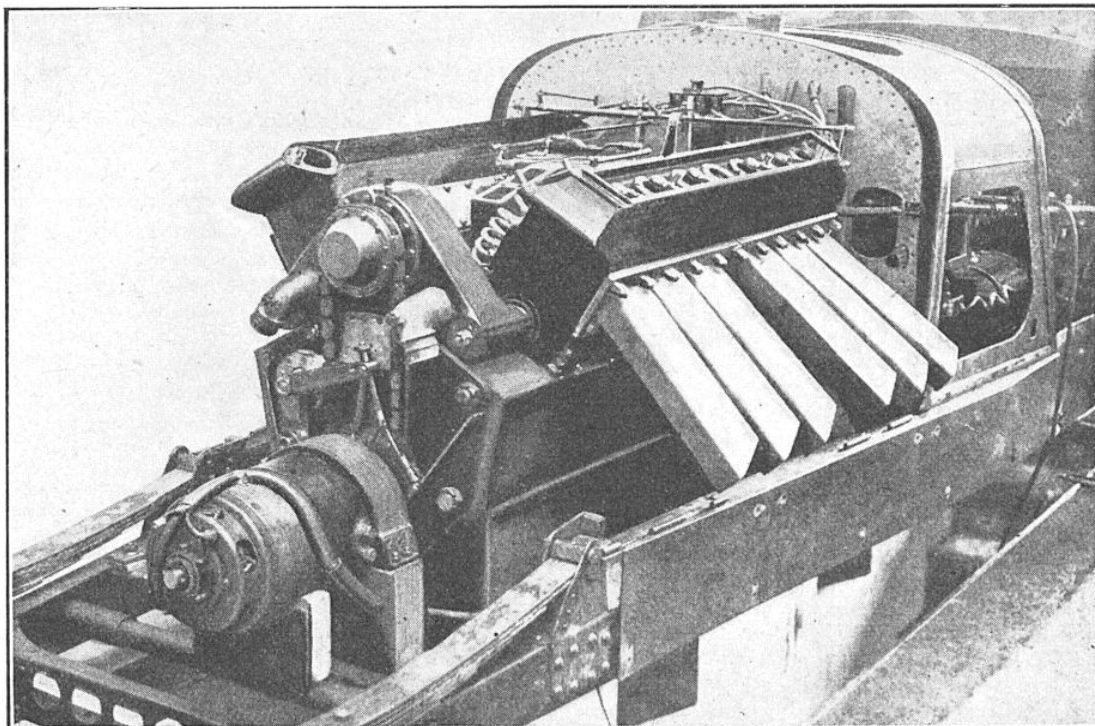
ENSEMBLE DU MOTEUR SANS SOUPAPES « VOISIN » 22 CH, 12 CYLINDRES EN V
