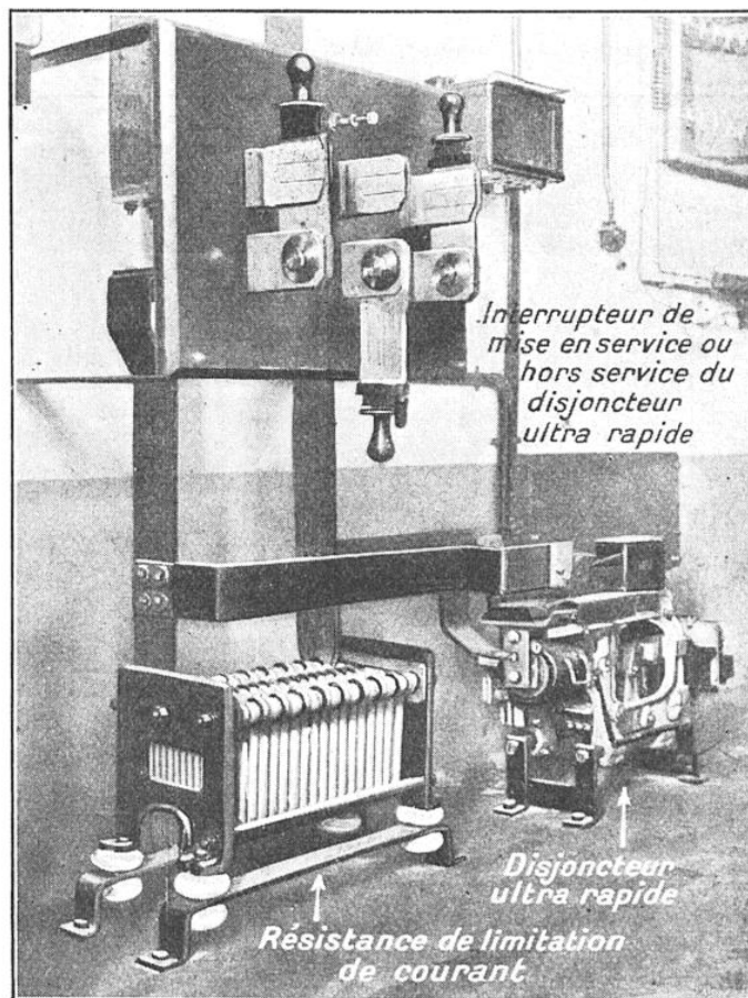
DISJONCTEUR AUTOMATIQUE ULTRA-RAPIDE COUPANT LE COURANT EN 1/100 e DE SECONDE
