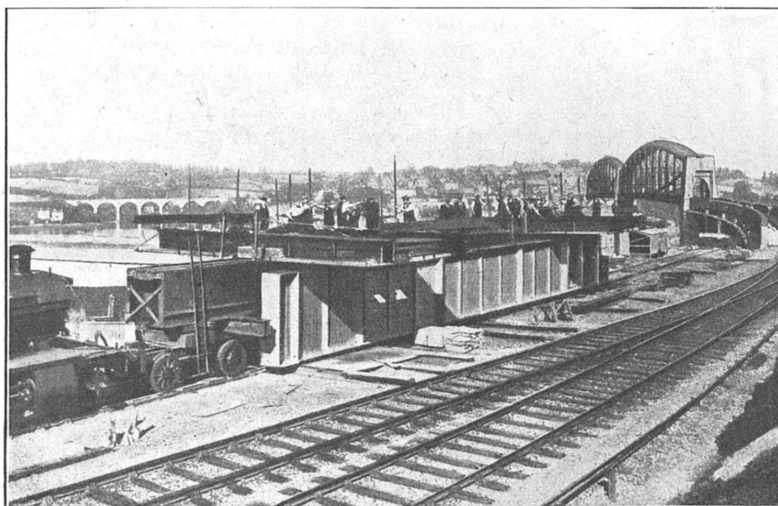
AU PREMIER PLAN, LE WAGON SPÉCIAL QUI A PERMIS DE REMPLACER LES TRAVERSES LONGITUDINALES ET TRANSVERSALES DU PONT SANS INTERROMPRE LE TRAFIC
