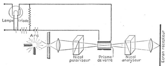
FIG. 11. — UN CURIEUX PROCÉDÉ DE MODULATION PAR LE « PHÉNOMÈNE DE KERR »
