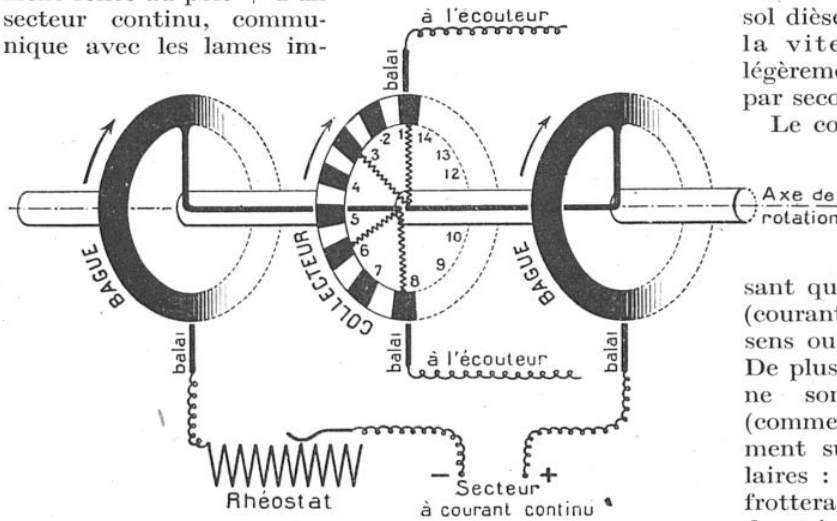
FIG. 11. — LE PLUS SIMPLE GÉNÉRATEUR ÉLECTROSONORE : LE COMMUTATEUR TOURNANT
