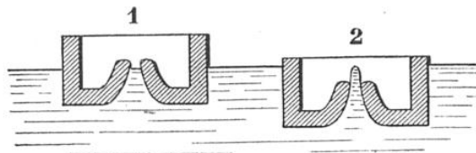
FIG. 10. — COUPE DE LA « DÉBITEUSE » UTILISÉE DANS LE PROCÉDÉ FOURCAULT
