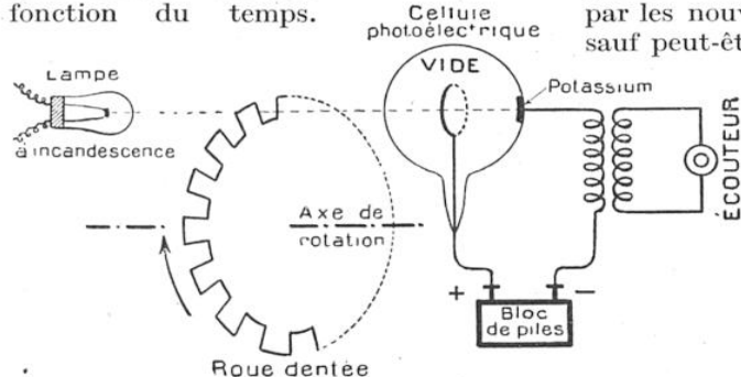
FIG. 16. — PRINCIPE D'UN INSTRUMENT PHOTOÉLECTRIQUE
