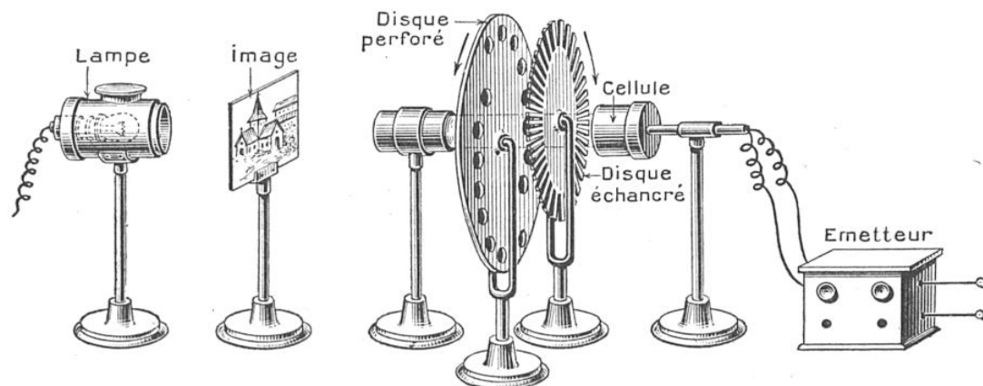
FIG. 12. — SCHÉMA DE L'ENSEMBLE DU DISPOSITIF DE TRANSMISSION DE BAIRD (QUI SE RETROUVE, INVERSÉ, A LA RÉCEPTION)
