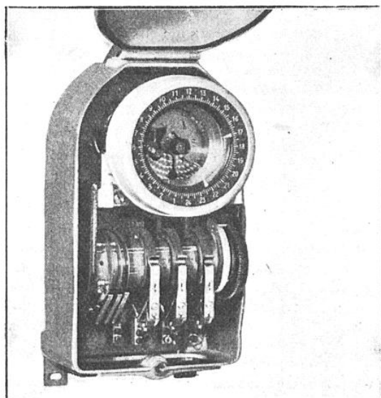
HORLOGE A CONTACTS POUR LA MISE EN SERVICE ET L'ARRÊT AUTOMATIQUES DE LA SOUS-STATION DU HOURAT (MIDI)
