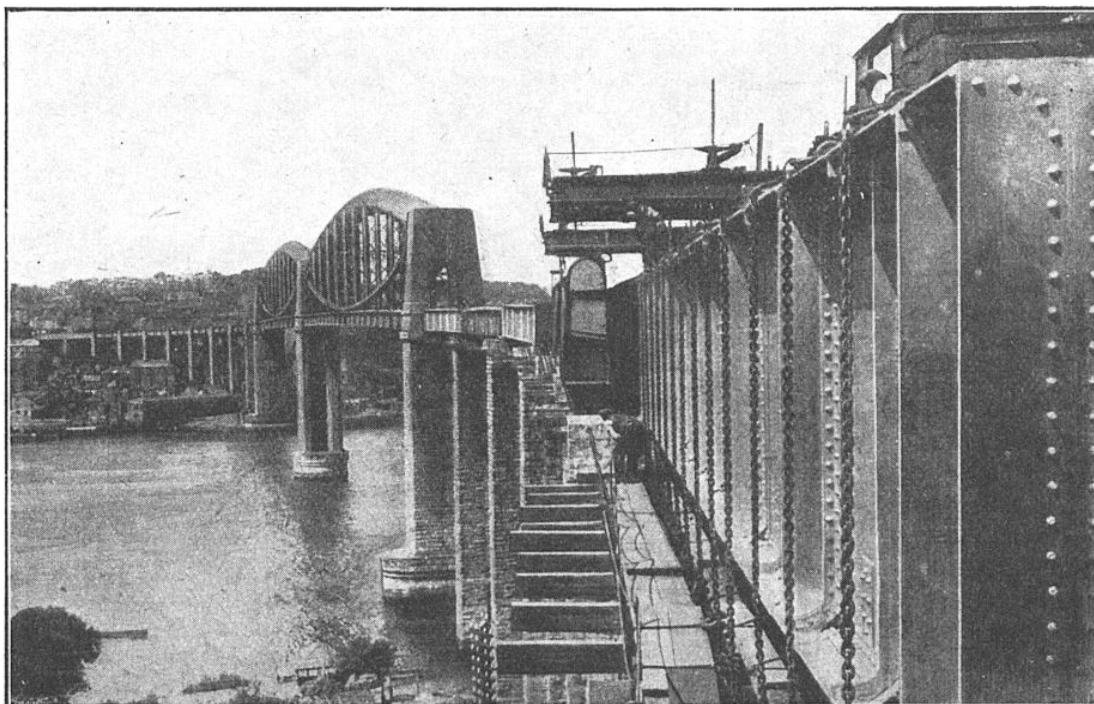
VUE D'ENSEMBLE DU PONT DU ROI-ALBERT A SALTASH (CORNOUAILLES) DONT LES ARCHES SITUÉES AU-DESSUS DU SOL VIENNENT D'ÊTRE RÉPARÉES SANS INTERROMPRE LE TRAFIC FERRÉ SUR CE PONT
