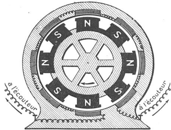
FIG. 12. — UN ALTERNATEUR A FRÉQUENCE MUSICALE
