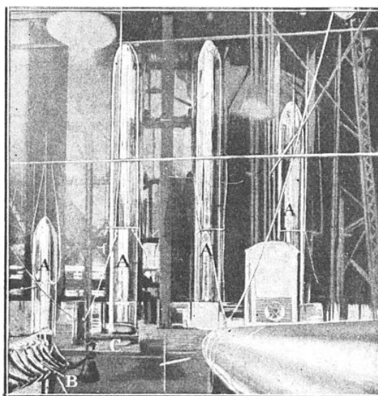
FIG. 4. — SALLE D'ÉTIRAGE DE CYLINDRES DE VERRE (PROCÉDÉ DE L'AMERICAN WINDOW GLASS)
