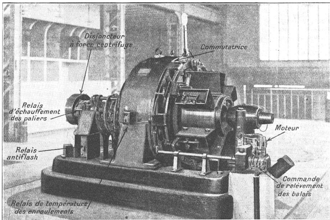
UNE DES MACHINES COMMUTATRICES UTILISÉES DANS LA SOUS-STATION DE SÈVRES, PRÈS DE PARIS (S. T. C. R. P.)
