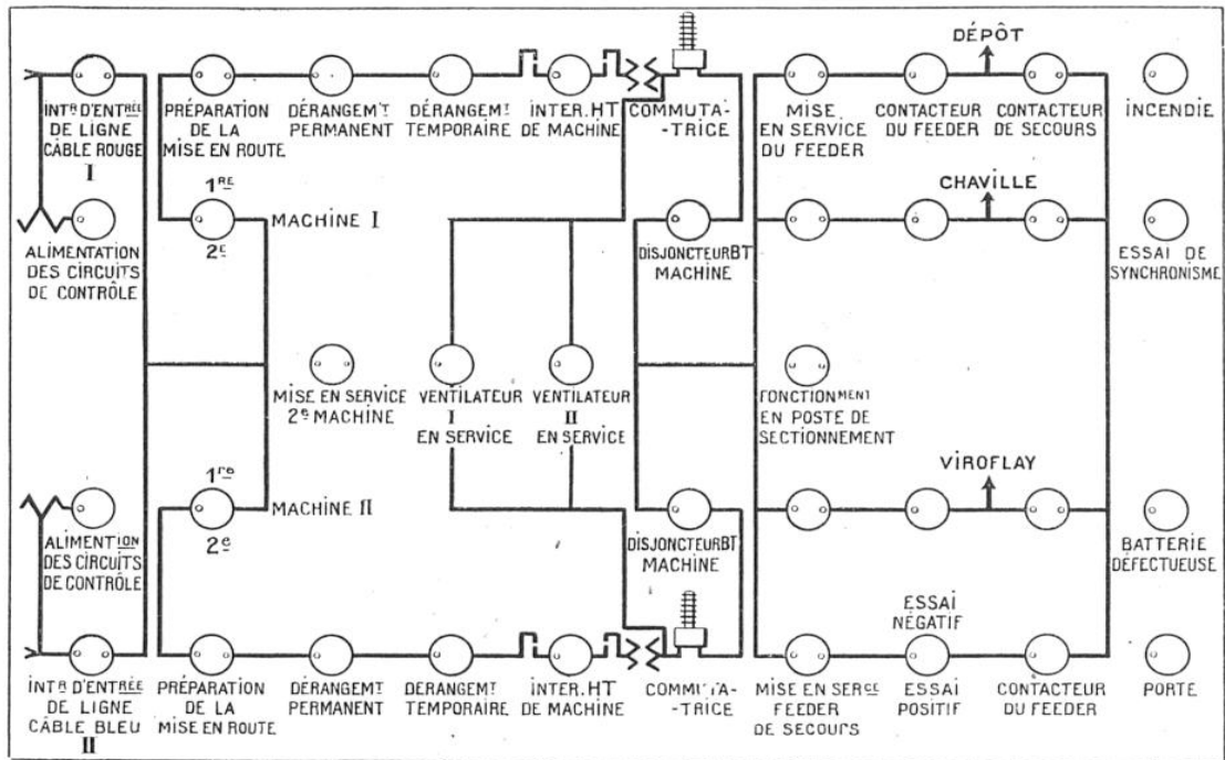
LE TABLEAU DE COMMANDE ET DE SIGNALISATION DE LA SOUS-STATION DE SÈVRES, TEL QUE L'OPÉRATEUR L'A DEVANT SES YEUX A « POINT-DU-JOUR »
