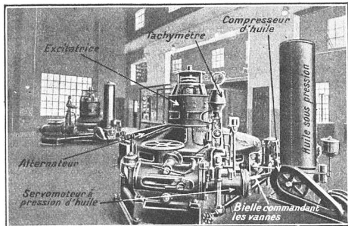
VUE INTÉRIEURE DE LA CENTRALE HYDROÉLECTRIQUE AUTOMATIQUE DE PINE-RIVER (ETATS-UNIS)
