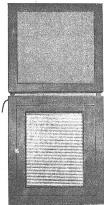
FIG. 5. — L'ÉCRAN RÉCEPTEUR AU NÉON DE LA BELL COMPANY
