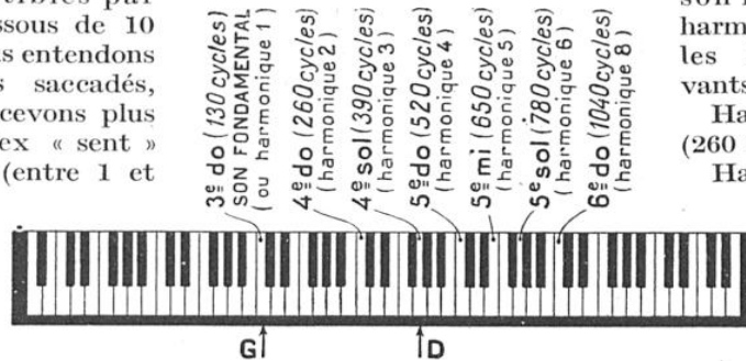
FIG. 6. — LES PRINCIPAUX HARMONIQUES D'UNE NOTE QUELCONQUE DU PIANO
