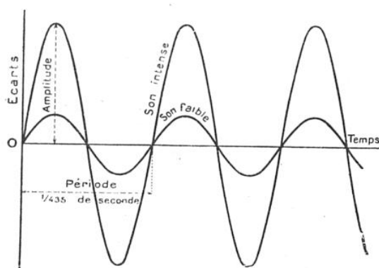
FIG. 1. — SONS FAIBLES ET SONS INTENSES.
