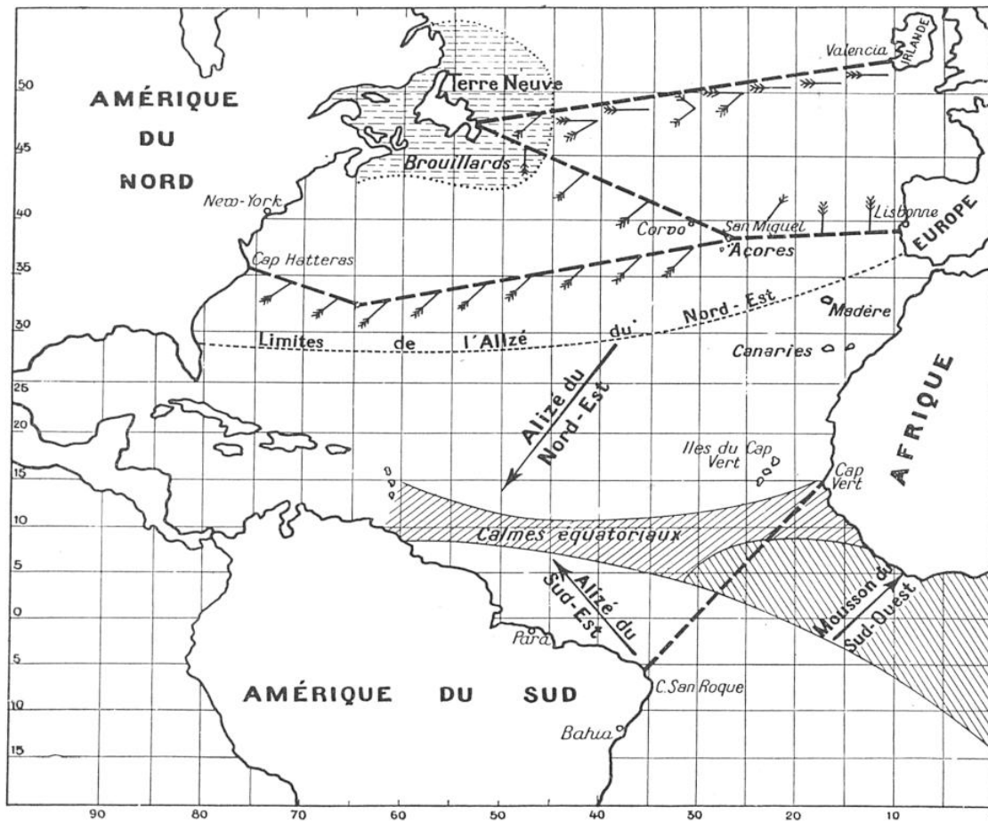
FIG. 5. — ÉTAT MOYEN DE L'ATMOSPHÈRE EN JUILLET DE CHAQUE ANNÉE SUR L'ATLANTIQUE. La direction du vent dominant, suivant les routes principales envisagées pour les traversées de l'Atlantique, est indiquée par une flèche, d'autant plus empennée qu'il est plus fort.
