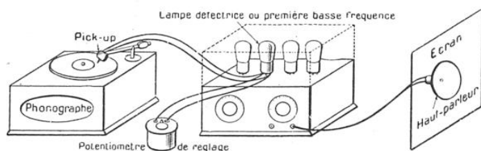
FIG. 1. — SCHÉMA D'UN DISPOSITIF DE REPRODUCTION POUR CINÉMATOGRAPHIE SONORE, RÉALISÉ À L'AIDE D'UN POSTE DE T. S. F. ORDINAIRE
