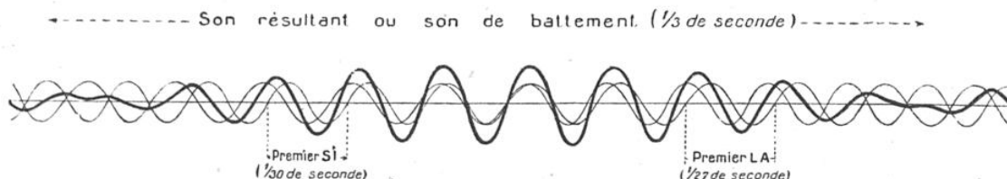
FIG. 14. — PRINCIPE DE L'HÉTÉRODYNE
