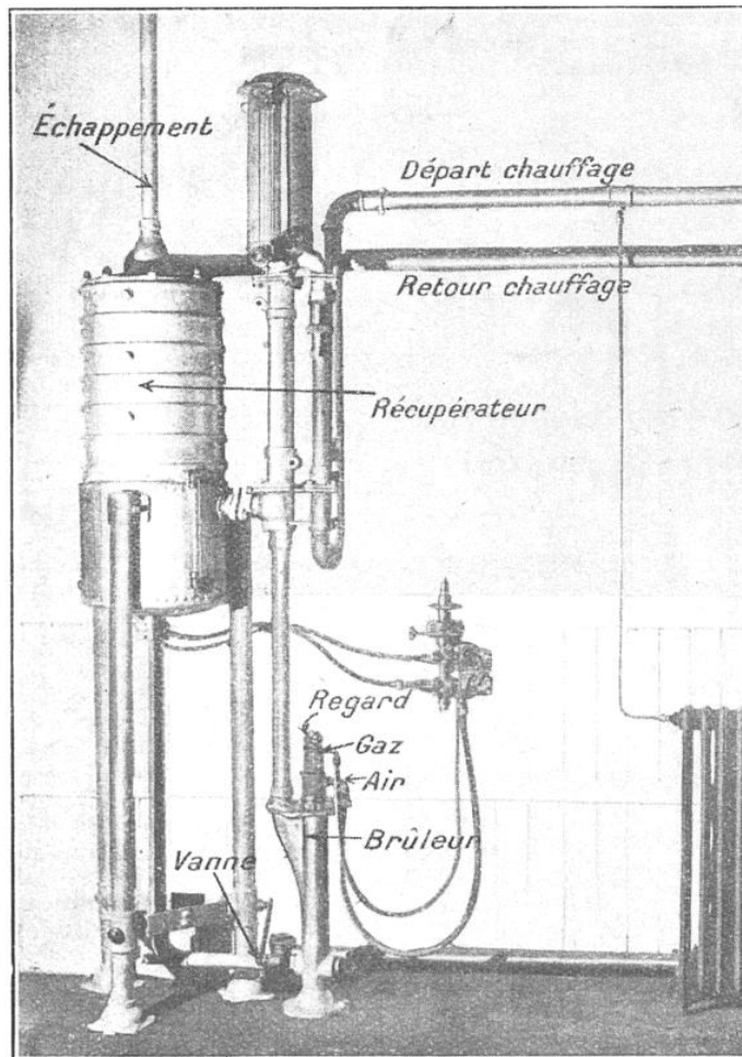
ENSEMBLE DE LA CHAUDIÈRE A GAZ « HAMMOND »
