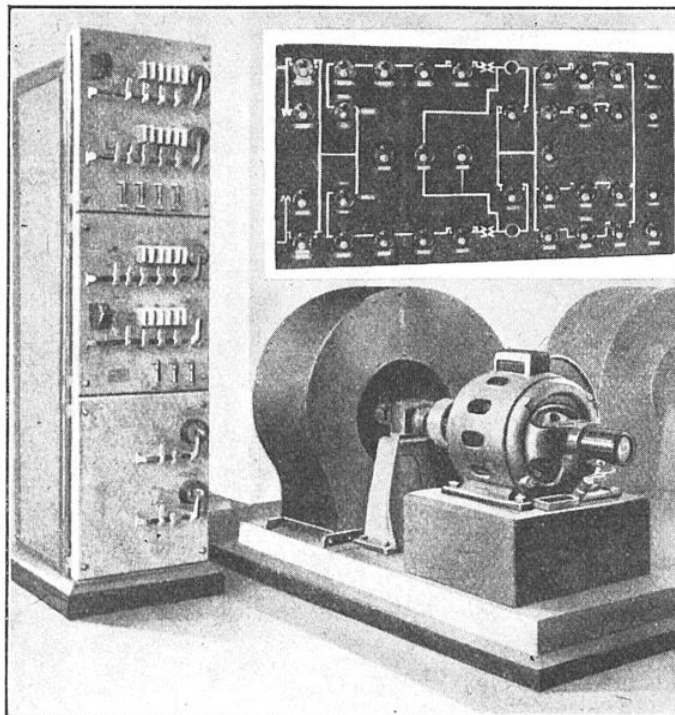
LE GROUPE DE VENTILATION DESTINÉ AU REFRIGÉRISEMENT DES TRANSFORMATEURS, DANS LA STATION DE SÈVRES, PRÈS DE PARIS, ET, A GAUCHE, SON PANNEAU DE DÉMARRAGE AUTOMATIQUE
