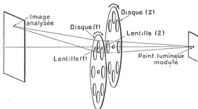
FIG. 9. — LES DISQUES ANALYSEURS DE M. BRILLOUIN
