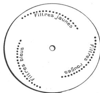
FIG. 8. — ROUE DE NIPKOW PERFECTIONNÉE PAR J. L. BAIRD EN VUE DE LA TÉLÉVISION COLORÉE
