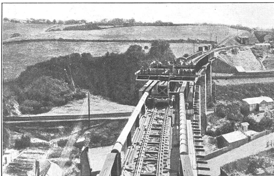
ENSEMBLE DES TRAVAUX PENDANT LA RÉPARATION DU PONT
