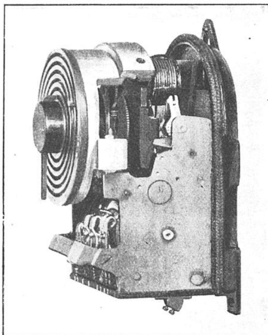
UN RELAIS « A ACTION DIFFÉRÉE »
