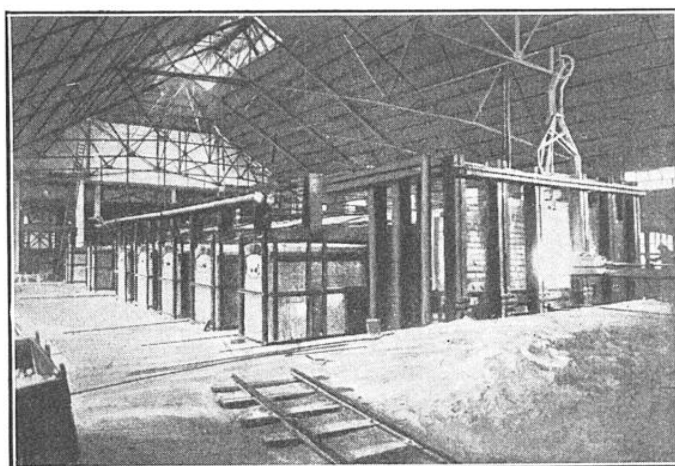
FIG. 8. — CHARGEMENT D'UN FOUR DE FUSION A BASSIN DANS LE PROCÉDÉ FOURCAULT
