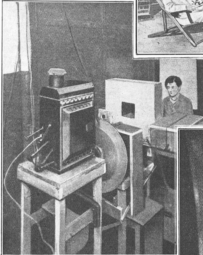
FIG. 13. — L'ÉCLAIRAGE DU SUJET PAR BALAYAGE D'UN RAYON LUMINEUX SURINTENSIFIÉ Le rayon est obtenu par concentration de la lumière d'un puissant projecteur électrique (enclos, ici, dans une lanterne). Au devant, la roue spirallée; entre le sujet et la lumière, un écran sert à régler l'aire de balayage.
