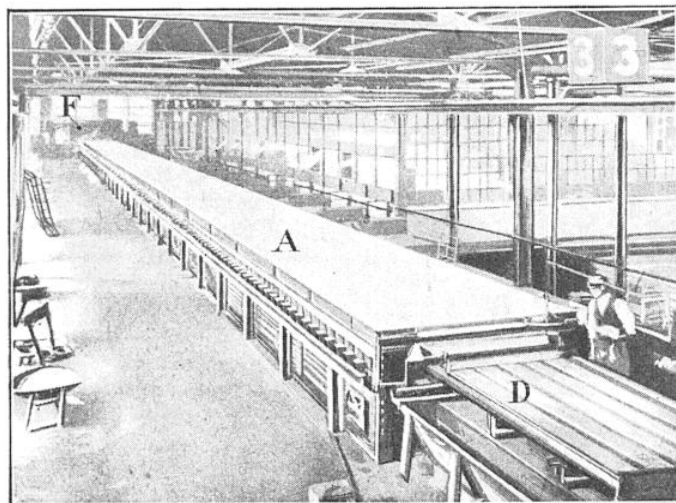
FIG. 13. — VUE D'ENSEMBLE D'UN HALL D'ÉTIRAGE POUR LA FABRICATION MÉCANIQUE DU VERRE À VITRE (PROCÉDÉ LIBBEY-OWENS)
