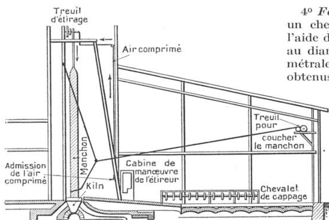
FIG. 5. — COUPE LONGITUDINALE D'UN ATELIER DE L'AMERICAN WINDOW GLASS, MONTRANT LE MANCHON DE VERRE TERMINÉ EN POSITION VERTICALE
