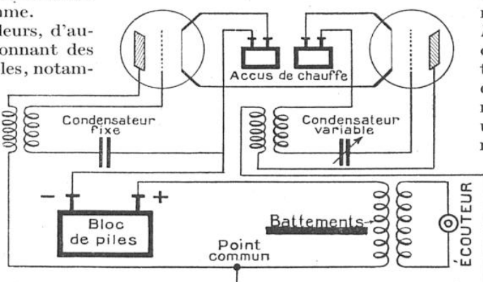
FIG. 15. — UN OSCILLATEUR HÉTÉRODYNE
