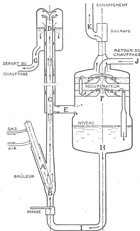
VUE EN COUPE DE LA CHAUDIÈRE «HAMMOND» A, brûleur ; B C D, échangeur-circulateur ; E F, entrée des gaz brûlés dans le récupérateur ; G, départ d'eau chaude ; H I, retour de l'eau à l'échangeur-circulateur ; J, retour de l'eau de chauffage ; K, échappement des gaz.
