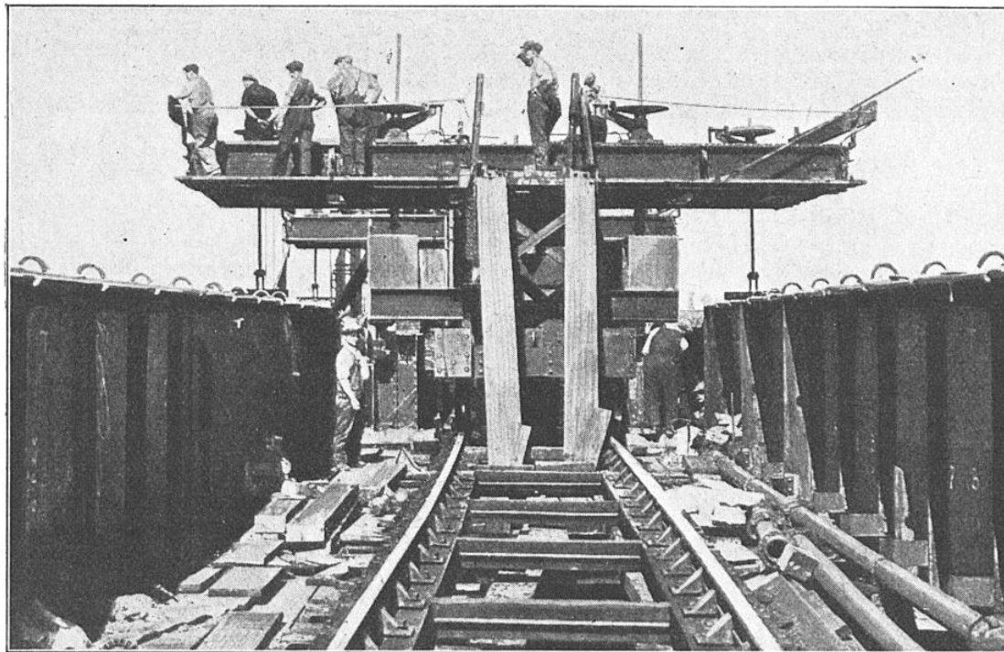
VUE EN BOUT DU WAGON SPÉCIAL UTILISÉ POUR LA RÉPARATION DU PONT DU ROI-ALBERT, A SALTASH (CORNOUAILLES)
