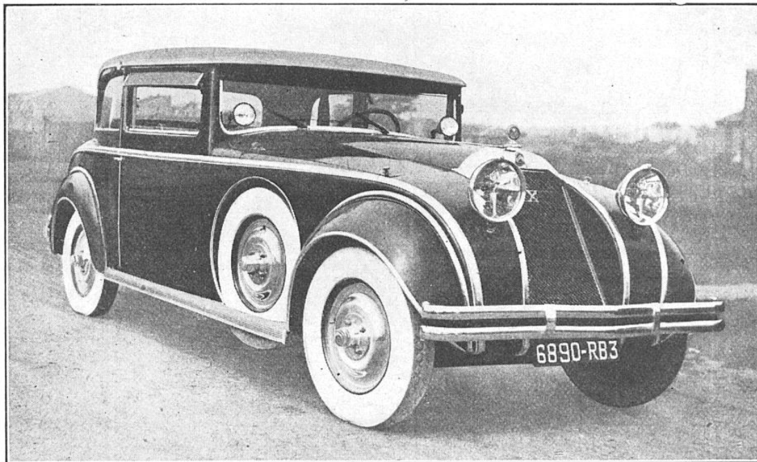
CETTE CARROSSERIE ORIGINALE, DÉBORDANT SUR LES ROUES, A PERMIS D'ÉLARGIR CONSIDÉRABLEMENT LA LARGEUR DE LA CAISSE, EN VUE D'AUGMENTER LE CONFORT
