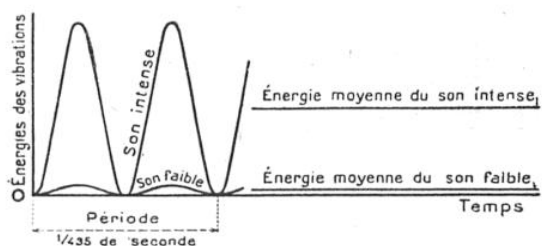
FIG. 2. — INTENSITÉ DES SONS
