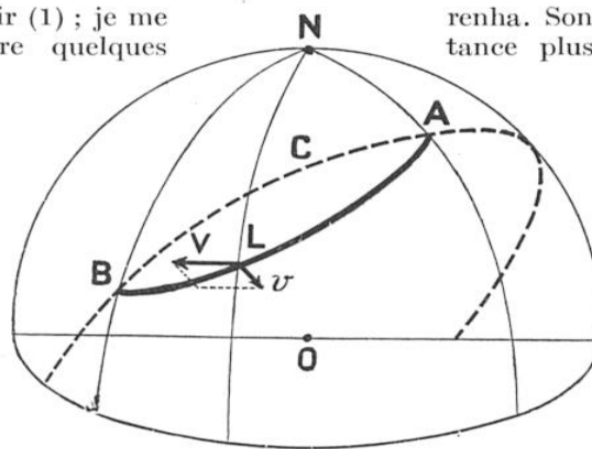
FIG. 6. — SCHÉMA DE LA ROUTE LA PLUS COURTE ENTRE A ET B SUR LA TERRE. ABC, grand coude ; ALB, loxodromie ; V, vitesse du vent ; v, vitesse de l'avion.
