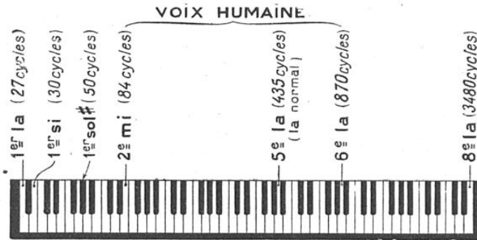
FIG. 4. — CLAVIER D'UN PIANO Avec les fréquences de quelques-unes des notes.
