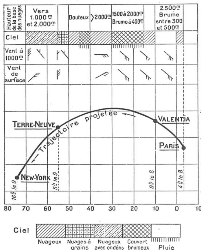
FIG. 4. — DIAGRAMME DU TEMPS PROBABLE POUR LES JOURNÉES DES 8 ET 9 MAI 1927, TEL QU'IL FUT DONNÉ A NUNGESSER ET COLI LE 7 MAI A 23 HEURES
