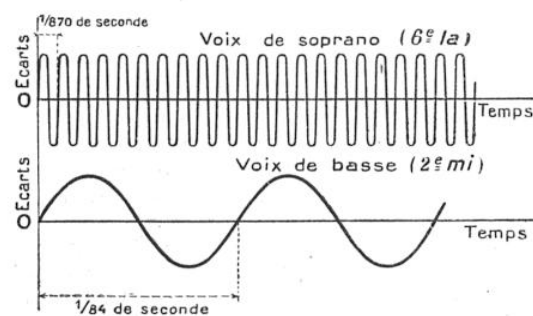
FIG. 3. — SONS AIGUS ET SONS GRAVES
