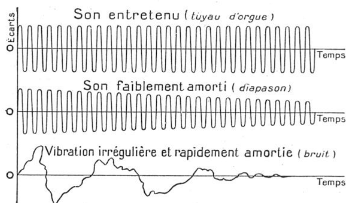
FIG. 8. — SONS ENTRETENUS ET SONS AMORTIS
