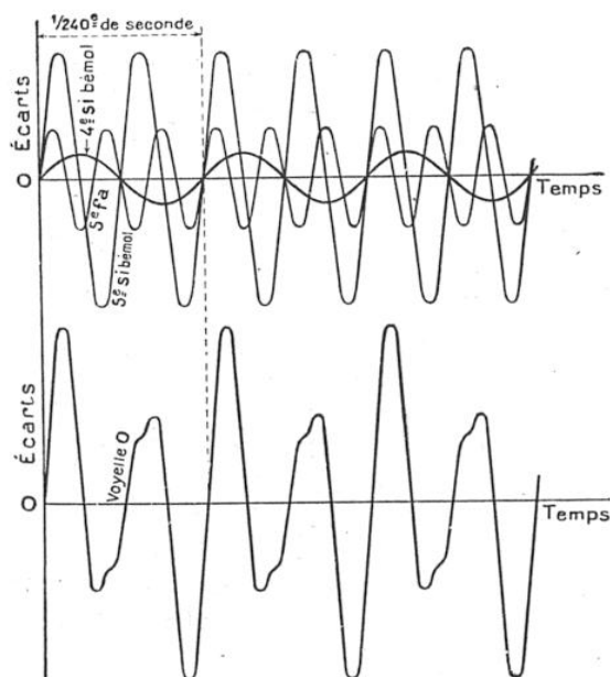
FIG. 7. — DE QUOI SE COMPOSE LE SON DE LA VOYELLE O
