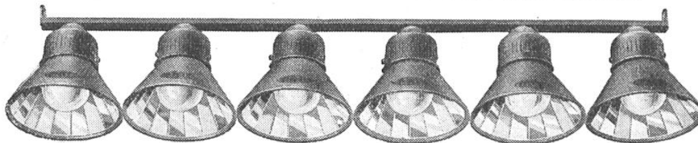
Rampe fixe n° 102, pour éclairage de vitrine, à raison de 6 éléments au mètre
