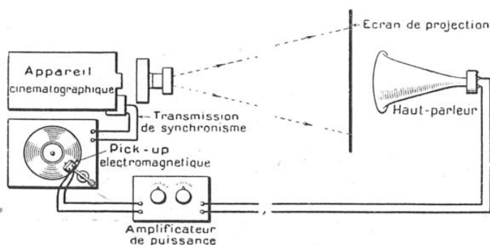
FIG. 2. — DISPOSITION SCHÉMATIQUE D'UN ENSEMBLE DE CINÉMATOGRAPHIE SONORE AVEC PHONOGRAPHE A REPRODUCTION ÉLECTRIQUE (POUR LA CLARTÉ DU DESSIN, LA FIGURE EST RÉDUITE EN LARGEUR)
