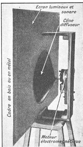
FIG. 5. — ÉCRAN LUMINEUX ET SONORE A MOTEUR ÉLECTROMAGNÉTIQUE RÉALISÉ PAR L'AUTEUR
