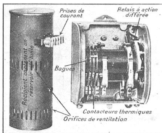
RELAIS D'ÉCHAUFFEMENT POUR PROTÉGER LES ALTERNATEURS
