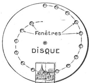
FIG. 7. — LA ROUE DE NIPKOW
