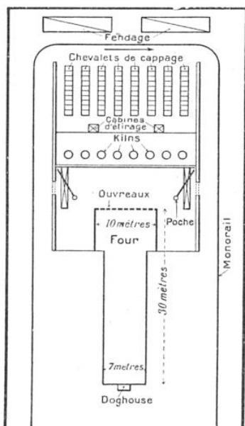
FIG. 6. — PLAN GÉNÉRAL DE LA VERRERIE A VITRES DE CHALON-SUR-SAONE (AMERICAN WINDOW GLASS)
