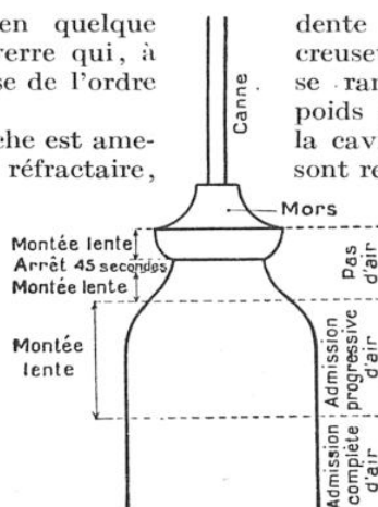
FIG. 3. — SCHÉMA D'ÉTIRAGE D'UN MANCHON DE VERRE (PROCÉDÉ DE L'AMERICAN WINDOW GLASS)
