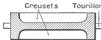
FIG. 2. — COUPE VERTICALE D'UN POT D'ÉTIRAGE, RÉVERSIBLE AUTOUR DE SES TOURILLONS
