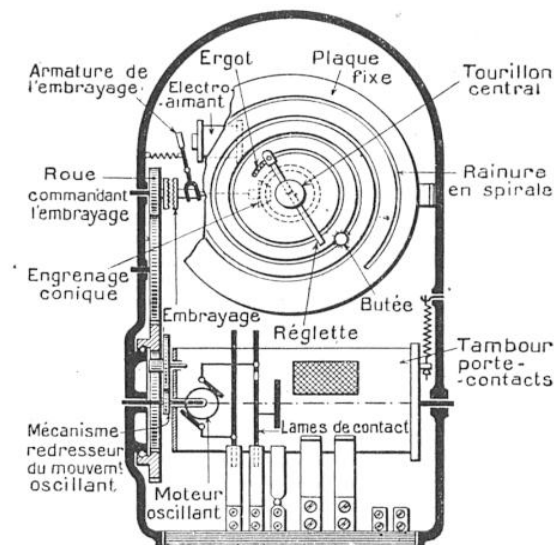
UN RELAIS « A ACTION DIFFÉRÉE »
