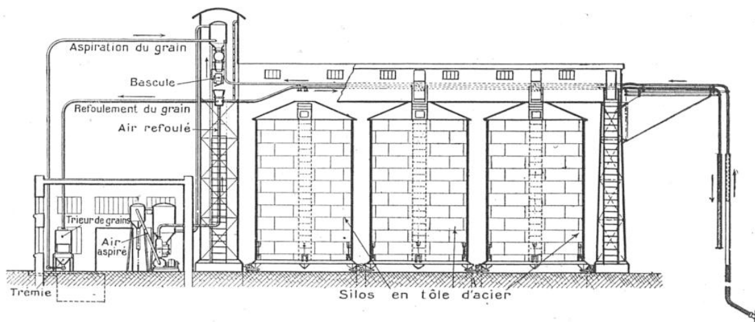
ENSEMBLE D'INSTALLATION D'UNE BATTERIE DE TROIS SILOS A GRAINS, AVEC MANUTENTION PNEUMATIQUE, D'UNE CAPACITÉ DE 500 TONNES
