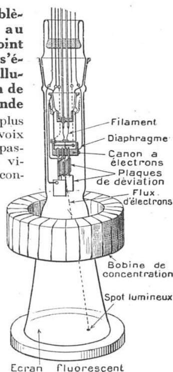
FIG. 4. — L'OSCILLOGRAPHIE CATHODIQUE TEL QUE M. DAUVILLIER L'A ADAPTÉ A SON « TÉLÉPHOTE »
