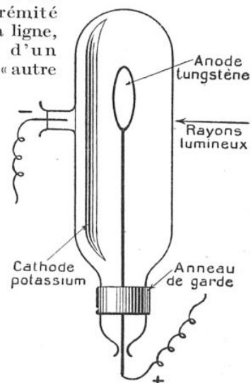
FIG. 2. — SCHÉMA DES CELLULES PHOTOÉLECTRIQUES GÉANTES ÉTABLIES PAR LES LABORATOIRES DE LA BELL COMPANY POUR RÉALISER SES DERNIERS TÉLÉVISEURS
