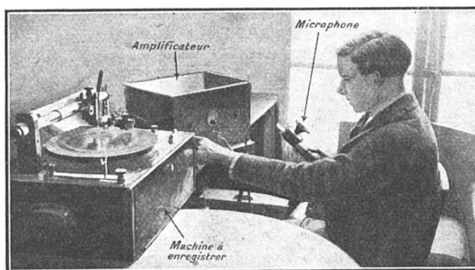
FIG. 4. — ESSAIS D'ENREGISTREMENT ÉLECTRIQUE DE LA PAROLE SUR DISQUE
