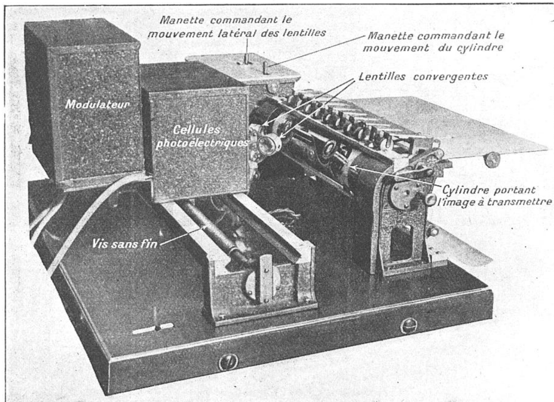
L'APPAREIL ÉMETTEUR SERVANT A L'EXPLORATION DU CLICHÉ DESTINÉ A ÊTRE TRANSMIS PAR T. S. F.
