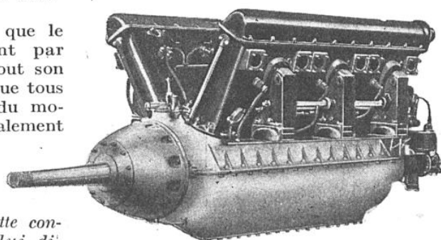
MOTEUR « HISPANO-SUIZA », 500 CH, 12 CYLINDRES NITRURÉS
