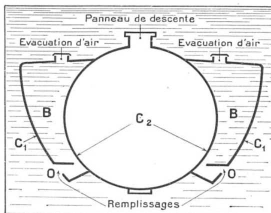
FIG. 1. — SECTION TRANSVERSALE D'UN SOUS-MARIN EN PLONGÉE, MONTRANT LA DISPOSITION DES WATER-BALLASTS
