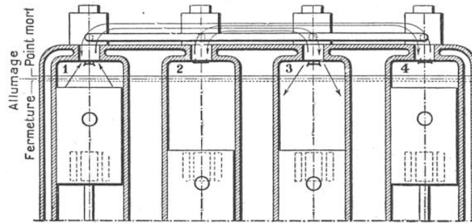
LE BRASSAGE DES GAZ CARBURÉS DANS LE MOTEUR « ROCHEFORT » (A DEUX TEMPS)
