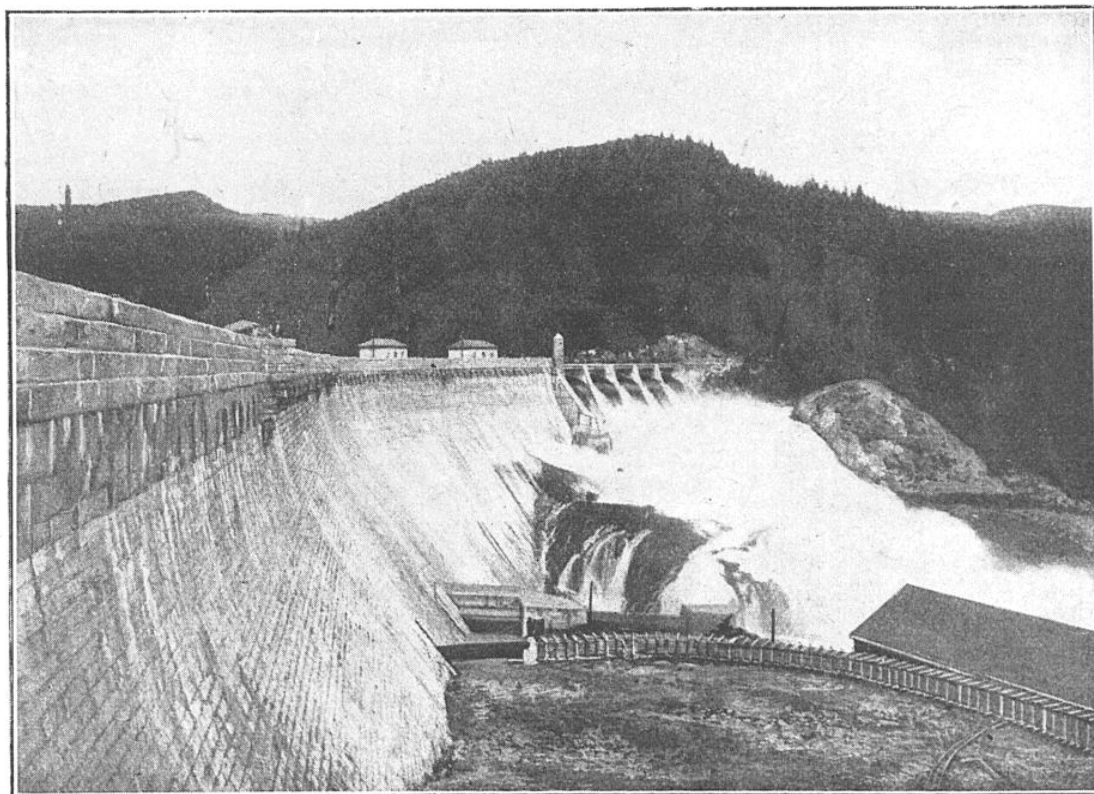
FIG. 3. — LE BARRAGE RÉGULATEUR DE DÉBIT, ÉTABLI A TUNHOVD, EN NUMEDAL (NORVÈGE), PERMET DE RETENIR 400 MILLIONS DE MÈTRES CUBES D'EAU
