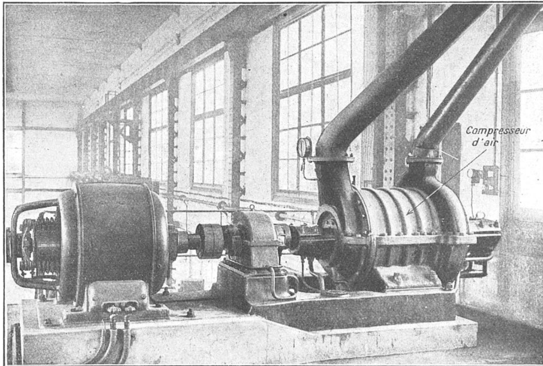
LABORATOIRE DES MOTEURS A ISSY-LES-MOULINEAUX (SEINE)
