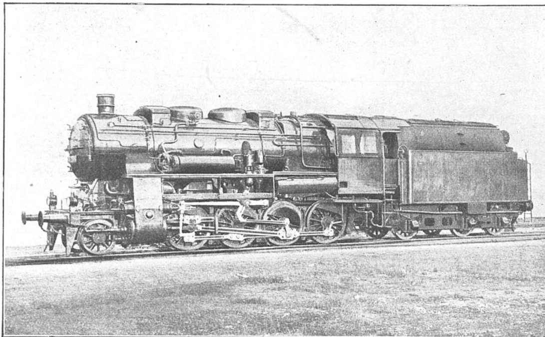
FIG. 1. — LA LOCOMOTIVE A CHARBON PULVÉRISÉ CONSTRUITE PAR L'A. E. G.
