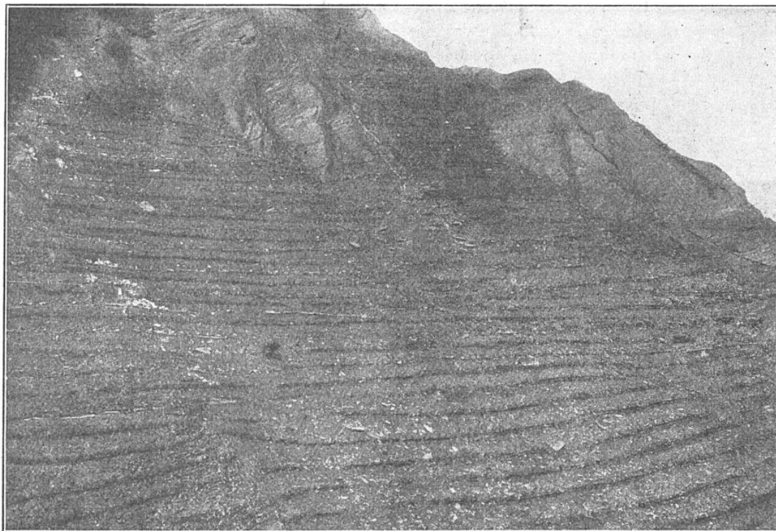
FIXATION, PAR DES CLAYONNAGES « VIVANTS », DU VERSANT DÉNUDÉ DU RAVIN DE L'EST, DANS LE TORRENT DES ROCHES NOIRES (SAVOIE)
