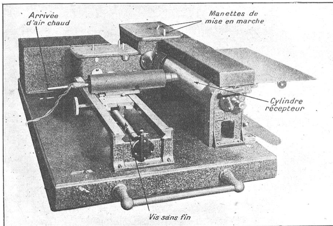
L'APPAREIL SERVANT A LA RÉCEPTION DES DOCUMENTS TRANSMIS PAR T. S. F.
