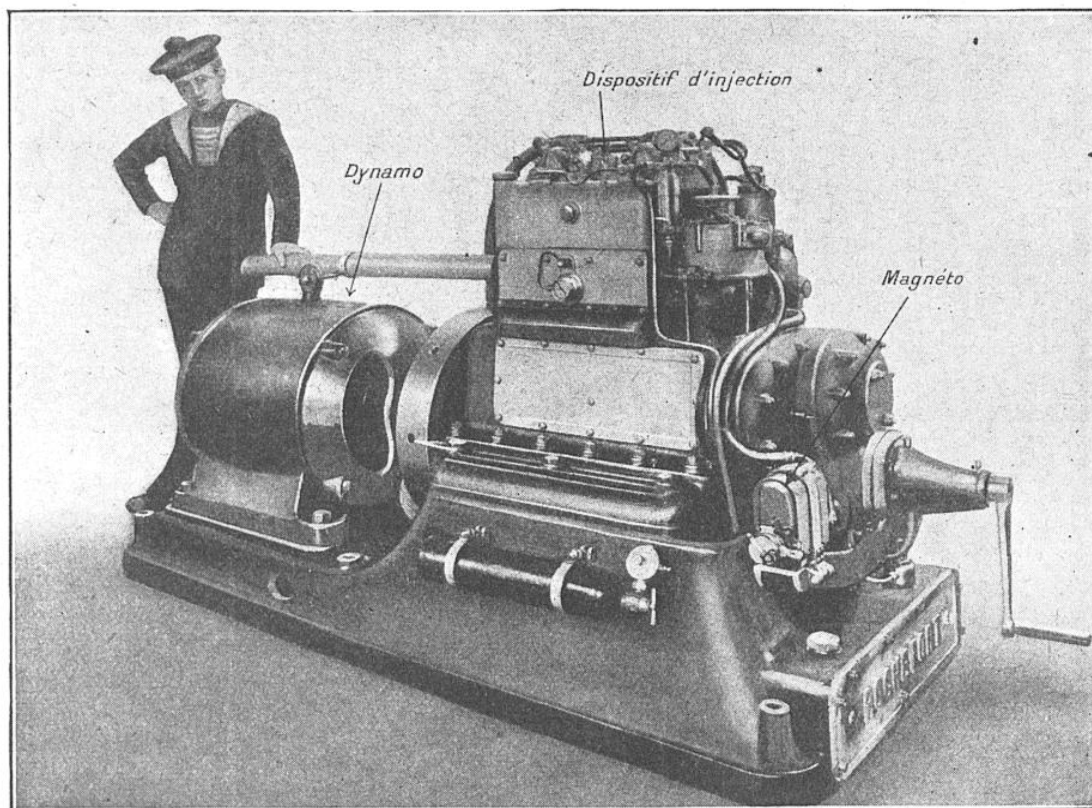
LE MOTEUR « ROCHEFORT » LÉGER, TYPE DE MARINE
