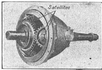
RÉDUCTEUR DE VITESSE POUR HÉLICE, SYSTÈME « FARMAN »
