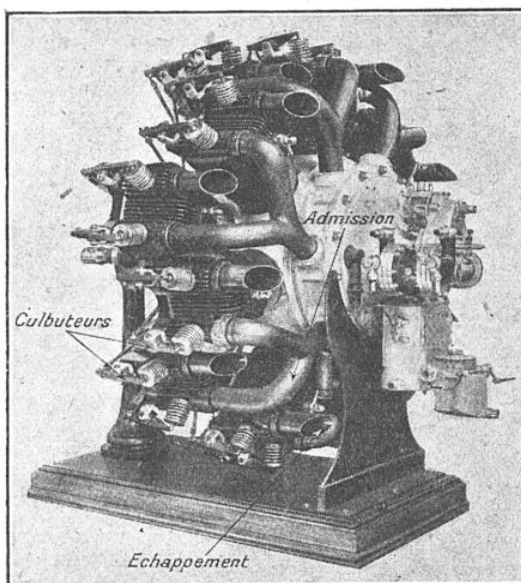
MOTEUR « LORRAINE », 430 CH, 14 CYLINDRES, EN DOUBLE ÉTOILE
