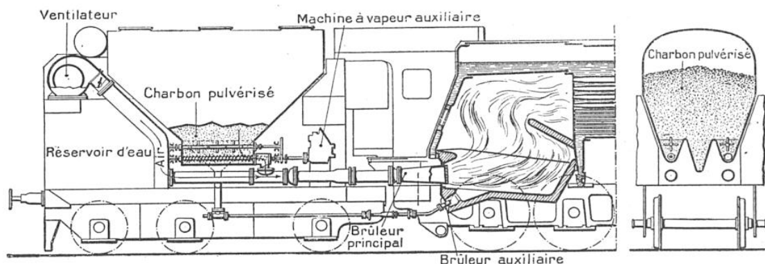
FIG. 2. — COUPE DU TENDER ET DU FOYER DE LA LOCOMOTIVE A CHARBON PULVÉRISÉ CONSTRUITS PAR LA « STUDIENGESELLSCHAFT »
