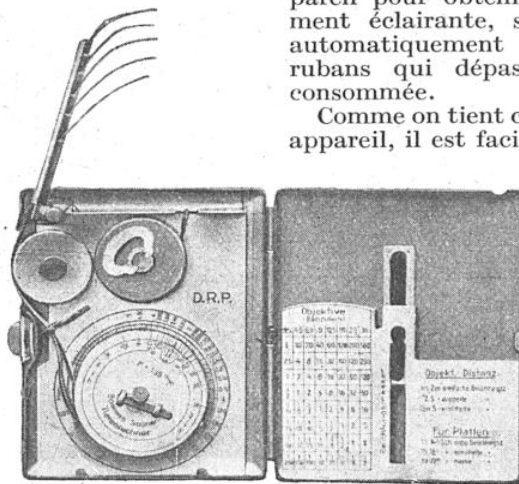
L'APPAREIL A CINQ RUBANS DE MAGNÉSIUM OUVERT
