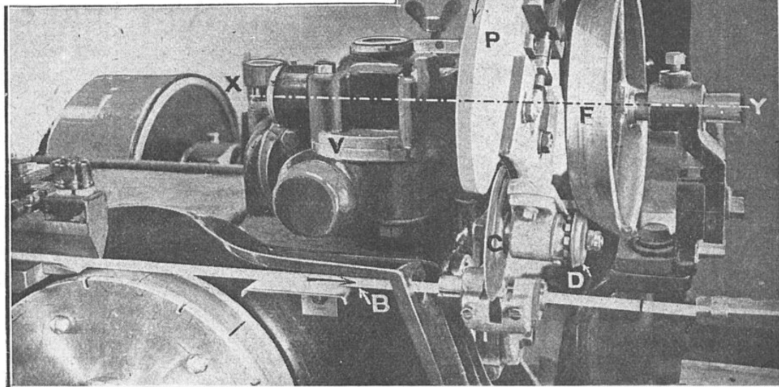
LA MACHINE « ASTRA » A TRANCHER LES CIGARETTES A LA LONGUEUR VOULUE
