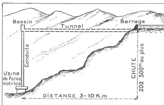
FIG. 2. — TYPE D'INSTALLATION DE CENTRALE HYDRAULIQUE ADOPTÉ EN NORVÈGE
