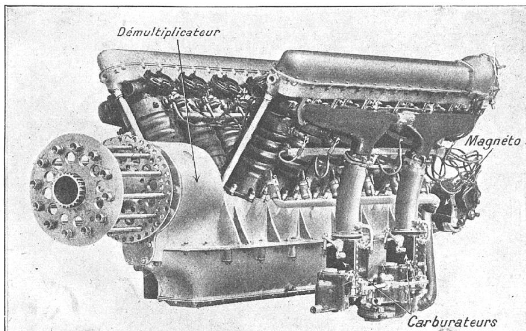
MOTEUR « RENAULT », 590 CH, 12 CYLINDRES EN V, AVEC DÉMULTIPLICATEUR A PRISE DIRECTE Les chemises de refroidissement par eau sont ondulées pour accroître le rayonnement thermique.
