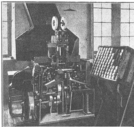
MACHINE, « SYSTÈME BELOT », A EMPAQUETER LE « SCAFERLATI »
