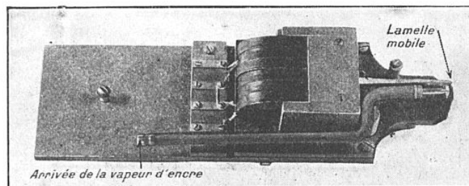
L'APPAREIL ENREGISTREUR A VAPEUR D'ENCRE DE R.-H. RANGER
