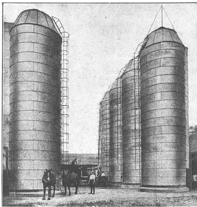
UNE BATTERIE DE HUIT SILOS A FOURRAGES S. I. M. A. Ces silos, d'une capacité de 170 mètres cubes chacun, assurent l'alimentation en fourrages d'un troupeau de deux cents vaches adultes (Société Agricole et Forestière de Chamthierry, à Saint-Maurice-le-Charancey, Orne).
