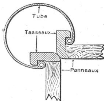
SCHÉMA DE JONCTION DE DEUX PANNEAUX DE BOIS AU MOYEN D'UN TUBE D'ACIER
