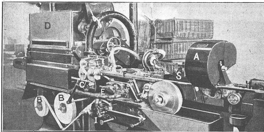
LA MACHINE AUTOMATIQUE « EXCELSIOR » A FABRIQUER LES CIGARETTES
