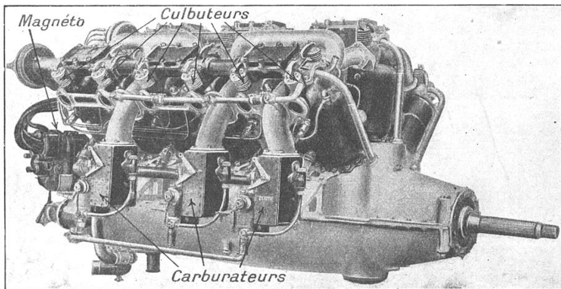
MOTEUR « LORRAINE », 400 CH, 12 CYLINDRES EN V
