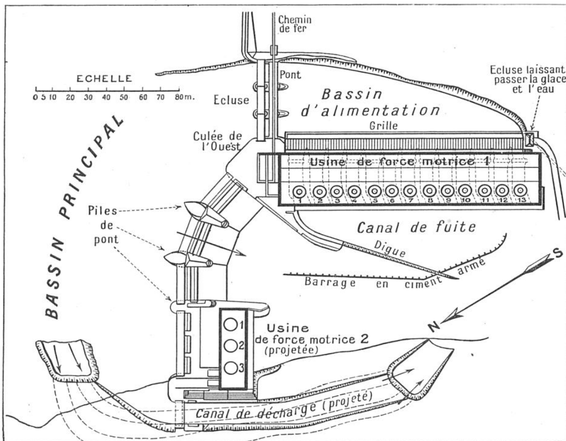
FIG. 6. — PLAN D'ENSEMBLE DE LA CENTRALE HYDRAULIQUE MØRKFOS-SOLBERGFOS (GLOMMEN), 149.500 CH
