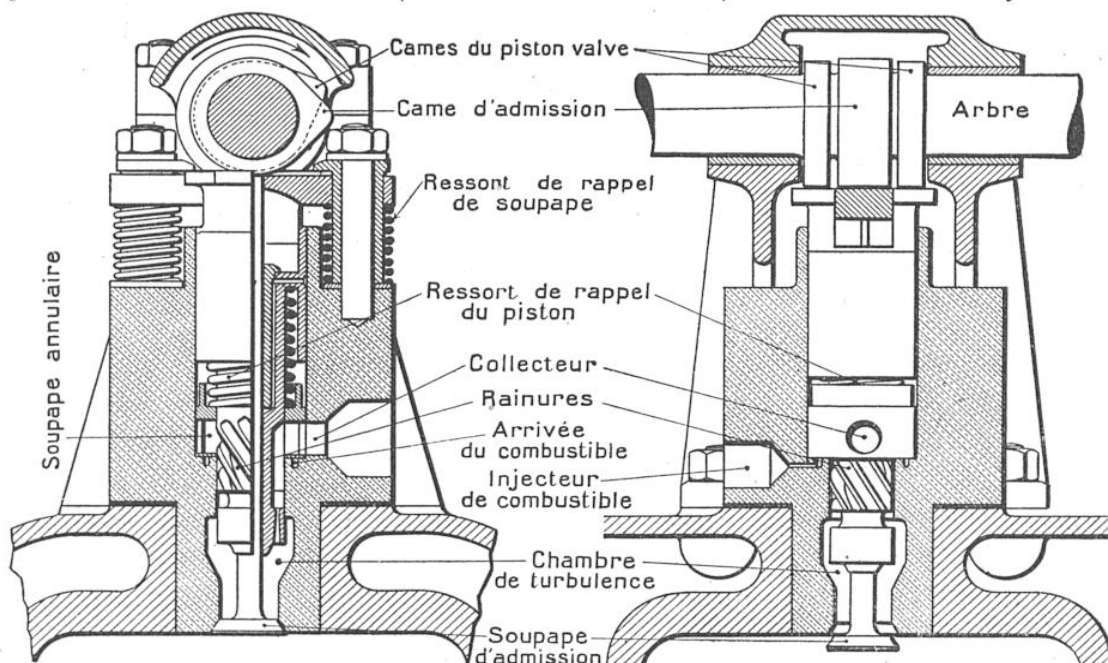
LE DISPOSITIF D'INJECTION DU MOTEUR « ROCHEFORT » A HUILE LOURDE
