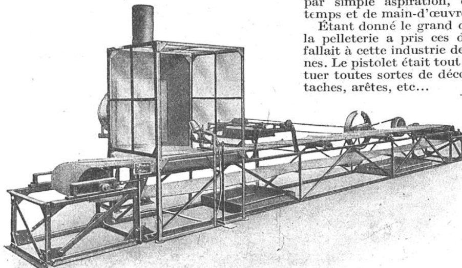
FIG. 3. — MACHINE AUTOMATIQUE POUR LA PEINTURE EN SÉRIE DE PLANCS D'ÉBÉNISTERIE
