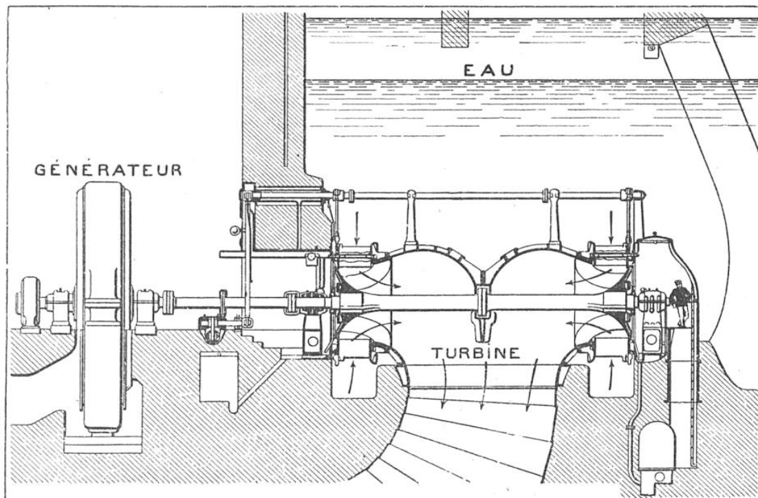
FIG. 4. — SCHÉMA D'UNE INSTALLATION D'UNE DES DOUZE TURBINES ET DU GÉNÉRATEUR ÉLECTRIQUE QU'ELLE ENTRAÎNE, A L'USINE DE RAANAASFOSS (72.000 CH)
