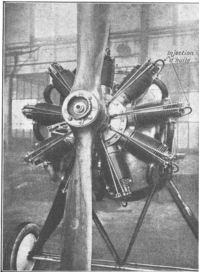
LE MOTEUR A HUILE LOURDE « CLERGET » (CYCLE DIESEL) Sans carburateur ni magnéto, ce moteur est la réplique française aux travaux similaires de Packard, en Amérique, et de Junkers, en Allemagne.
