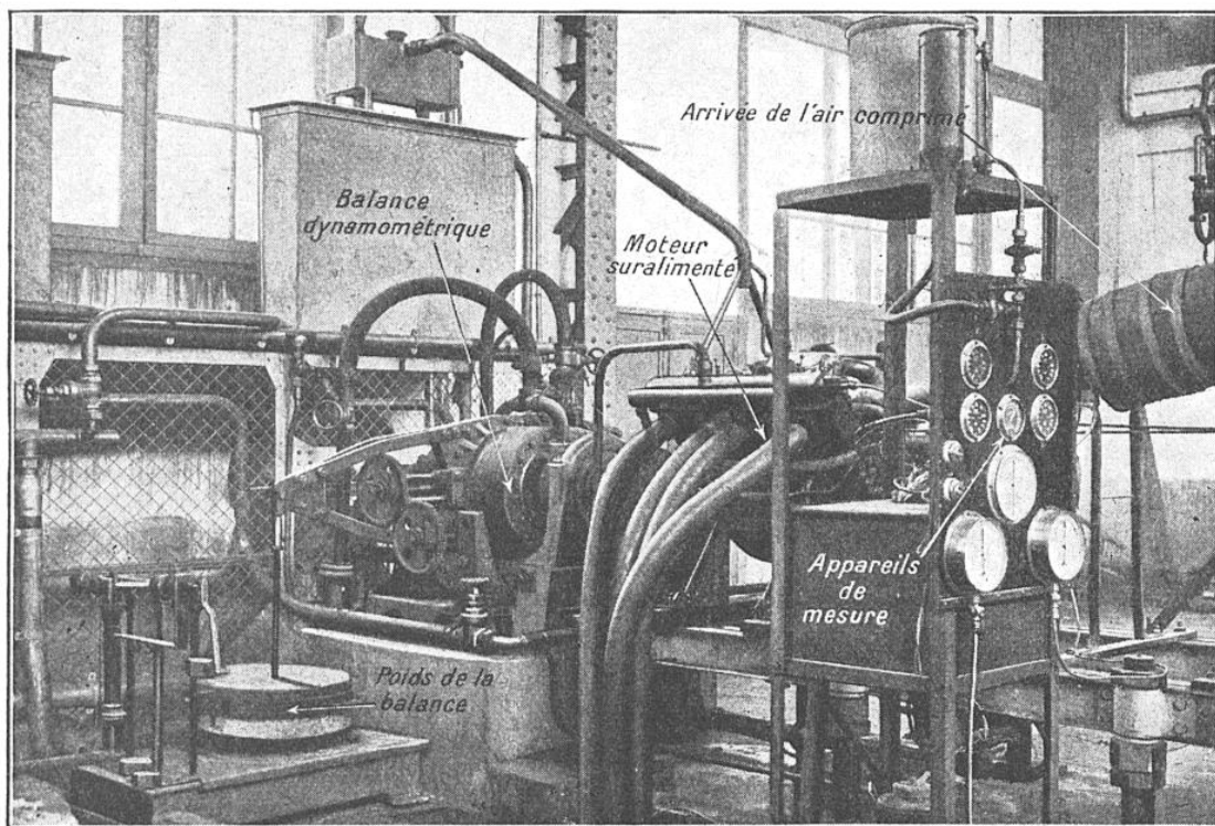
LABORATOIRE D'ESSAIS DES MOTEURS D'ISSY-LES-MOULINEAUX (SEINE)
