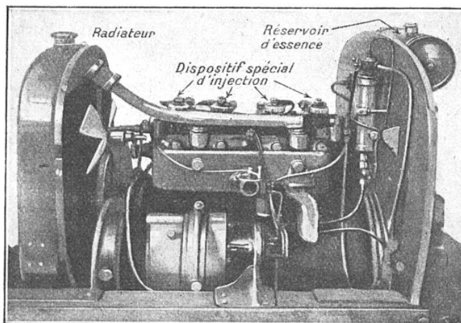
LE MOTEUR « ROCHEFORT » (A HUILE LOURDE) TEL QU'IL FONCTIONNAIT DÈS 1923 SUR UN CHASSIS D'AUTOMOBILE (VOIR SCHÉMA CI-DESSOUS)
