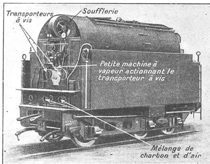
FIG. 3. — LE TENDER POUR LOCOMOTIVE A CHARBON PULVÉRISÉ CONSTRUITE PAR L'A. E. G.
