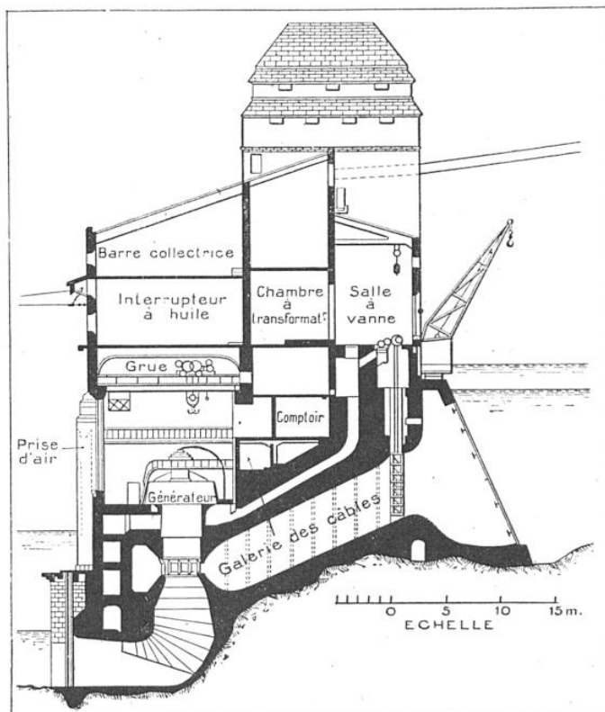
FIG. 7. — COUPE VERTICALE DE L'USINE MØRKFOS-SOLBERGFOS (GLOMMEN), 149.500 CH
