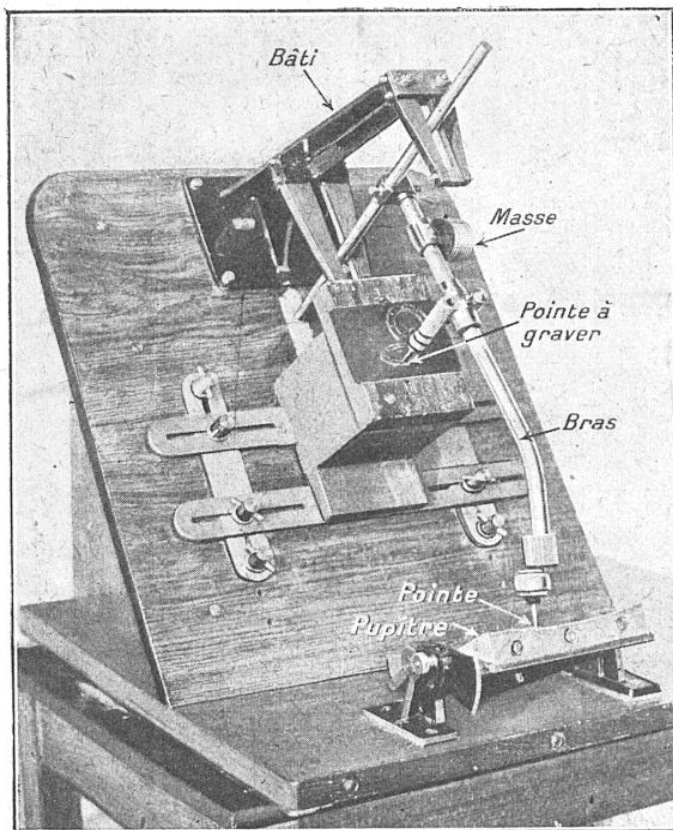
SUIVANT L'INCLINAISON DU PUPITRE SUR LEQUEL EST FIXÉ LE MODÈLE, LA POINTE À TRACER GRAVE UNE REPRODUCTION DÉFORMÉE DANS LE SENS DE LA HAUTEUR OU DE LA LARGEUR
