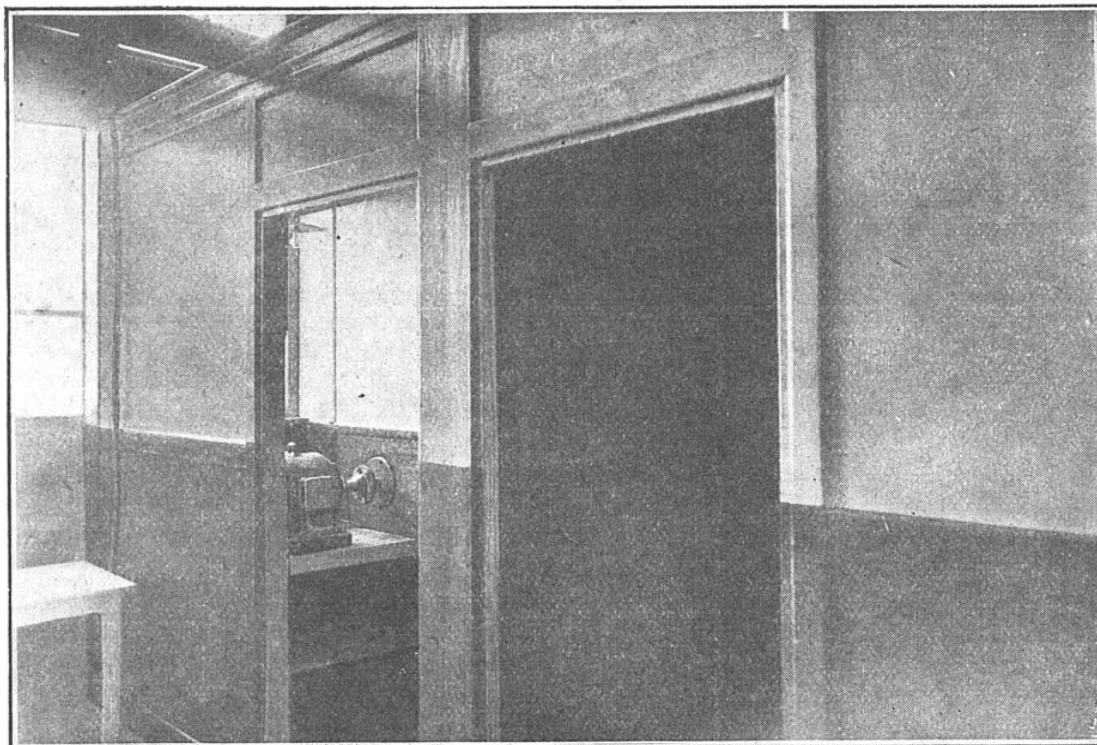
VOICI UNE DES CABINES D'ESSAI DE BOITES DE VITESSES, RENDUE SILENCIEUSE PAR L'INTERPOSITION D'UNE COUCHE D'« INSULITE » DANS LE PLAFOND ET LE PLANCHER, ET DE DEUX COUCHES DANS LES PAROIS
