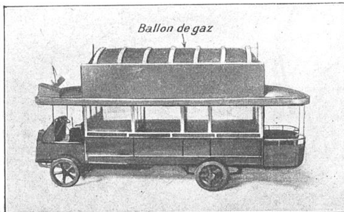
UN AUTOBUS PARISIEN FONCTIONNANT AU GAZ, PENDANT LA GUERRE
