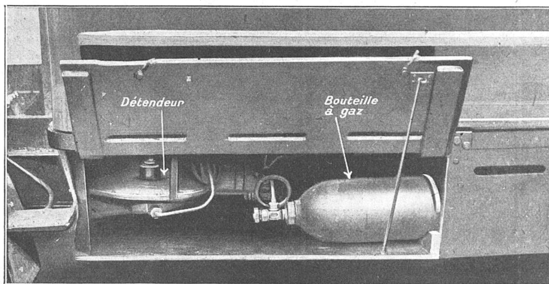
L'INSTALLATION DU DÉTENDEUR ET DES BOUTEILLES DANS LES CAISSONS DE L'AUTOBUS DE LA T. C. R. P. REPRÉSENTÉ SUR LA PAGE CI-CONTRE
