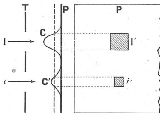
FIG. 5. — LA COURBE « CC' » INDIQUE LA RÉPARTITION LUMINEUSE SUR LA PLAQUE « P » SUIVANT L'INTENSITÉ LUMINEUSE I OU i TRAVERSANT LA TRAME « T ». IL EN RÉSULTE DES TACHES CLAIRES I' OU i' DE SURFACES DIFFÉRENTES
