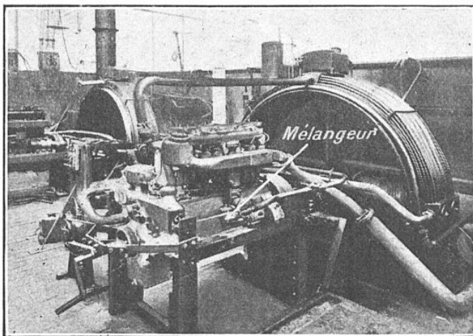
L'ESSAI AU BANC DE MOTEURS A EXPLOSIONS, NORMALEMENT ÉTABLIS POUR FONCTIONNER AVEC DES CARBURANTS LIQUIDES, ET ALIMENTÉS AU GAZ, A DONNÉ D'EXCELLENTS RÉSULTATS
