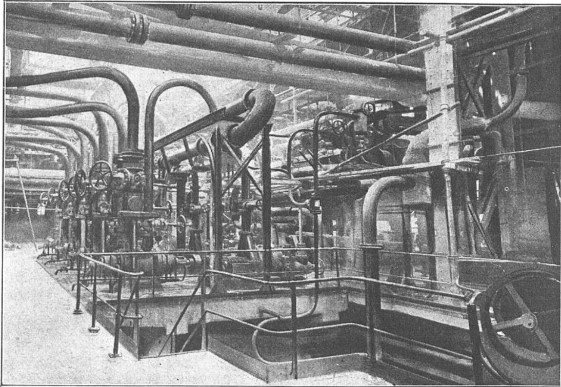
ENSEMBLE DES POMPES ALIMENTAIRES ET DES TUYAUTERIES D'ALIMENTATION DES CHAUDIÈRES D'ISSY-LES-MOULINEAUX
