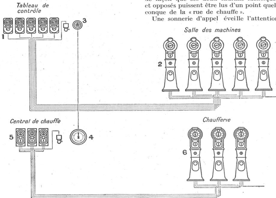
FIG. 8. — PLAN SCHÉMATIQUE D'UNE INSTALLATION-TYPE DE TRANSMISSION D'ORDRES A DISTANCE DANS UNE CENTRALE ÉLECTRIQUE
