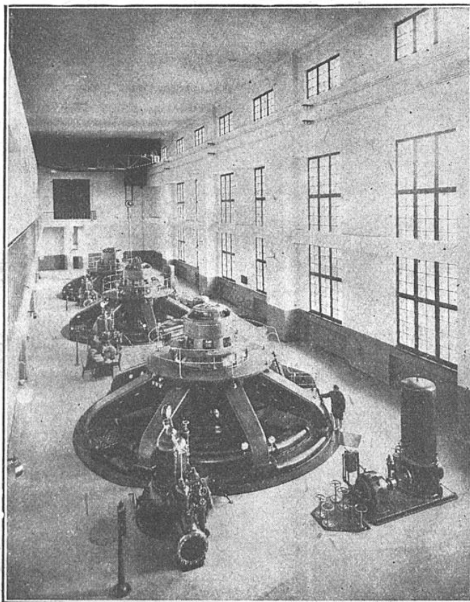
LES TURBINES VERTICALES FRANCIS DE 27.000 CH A L'USINE HYDROÉLECTRIQUE D'IMATRA
