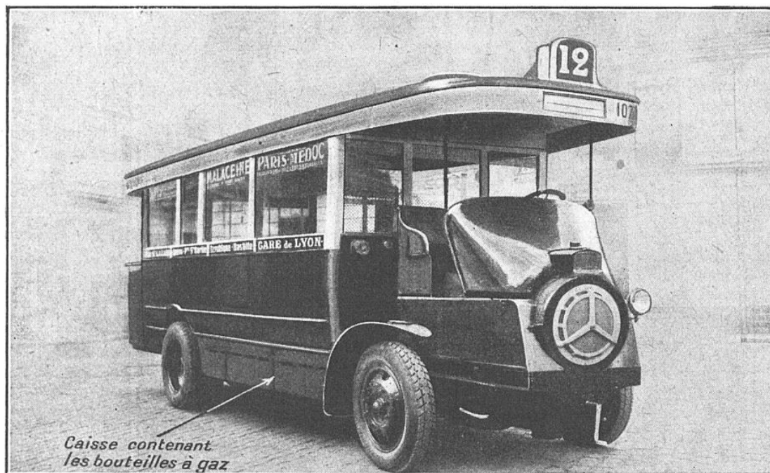
UN DES AUTOBUS A GAZ ACCOMPLISSANT AUJOURD'HUI LE SERVICE COURANT DE LA T. C. R. P.
