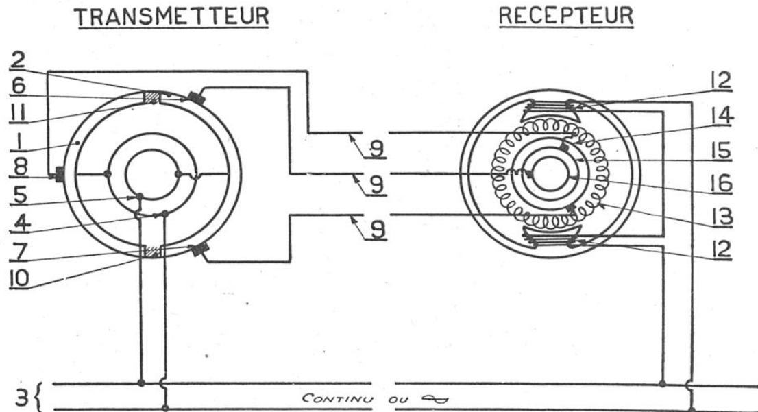
FIG. 1. — SCHÉMA DE L'APPAREIL TRANSMETTEUR-RÉCEPTEUR D'ORDRES A DISTANCE A NOMBRE DE POSITIONS LIMITÉ (SYSTÈME SAINT-CHAMOND-GRANAT)
