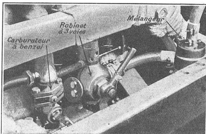
LE DISPOSITIF COMPLET D'ALIMENTATION D'UN DES AUTOBUS AU GAZ EN SERVICE A PARIS
