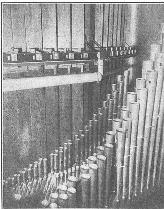
VUE PARTIELLE DES LAMES QUI CONSTITUENT LA « BOITE EXPRES- SIVE » DE L'ORGUE A TRANSMISSION ÉLECTROPNEUMATIQUE, CONSTRUIT PAR CAVAILLÉ COLL
