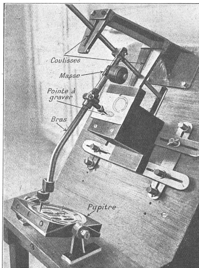
ENSEMBLE DU « PANGRAFIC » INDUSTRIEL
