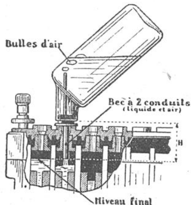
COMMENT ON UTILISE LE « NIVOSTOP » POUR LE REM- PLISSAGE DES ACCUMULATEURS
