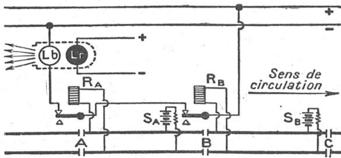
COMMENT FONCTIONNE EN PRINCIPE LE BLOC AUTOMATIQUE PAR « CIRCUITS DE VOIE »
