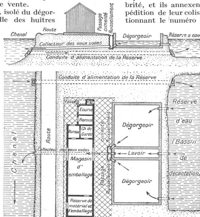
FIG. 6. — COUPE ET PLAN SCHÉMATIQUES D'UNE INSTALLATION-TYPE D'OSTRÉICULTURE
