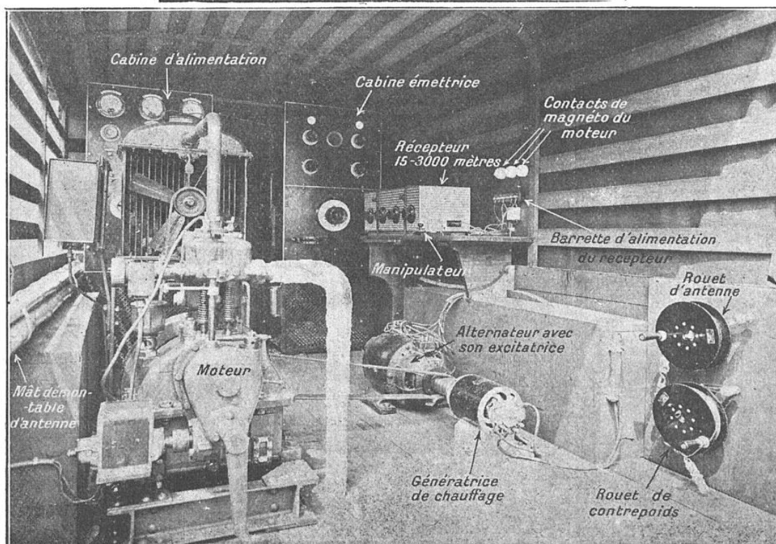
VUES EXTÉRIEURE ET INTÉRIEURE DE LA CAMIONNETTE « RADIO L.-L. », QUI A SERVI À MAINTENIR LA LIAISON RADIOTÉLÉGRAPHIQUE ENTRE LE « TOUR DE FRANCE » ET PARIS
