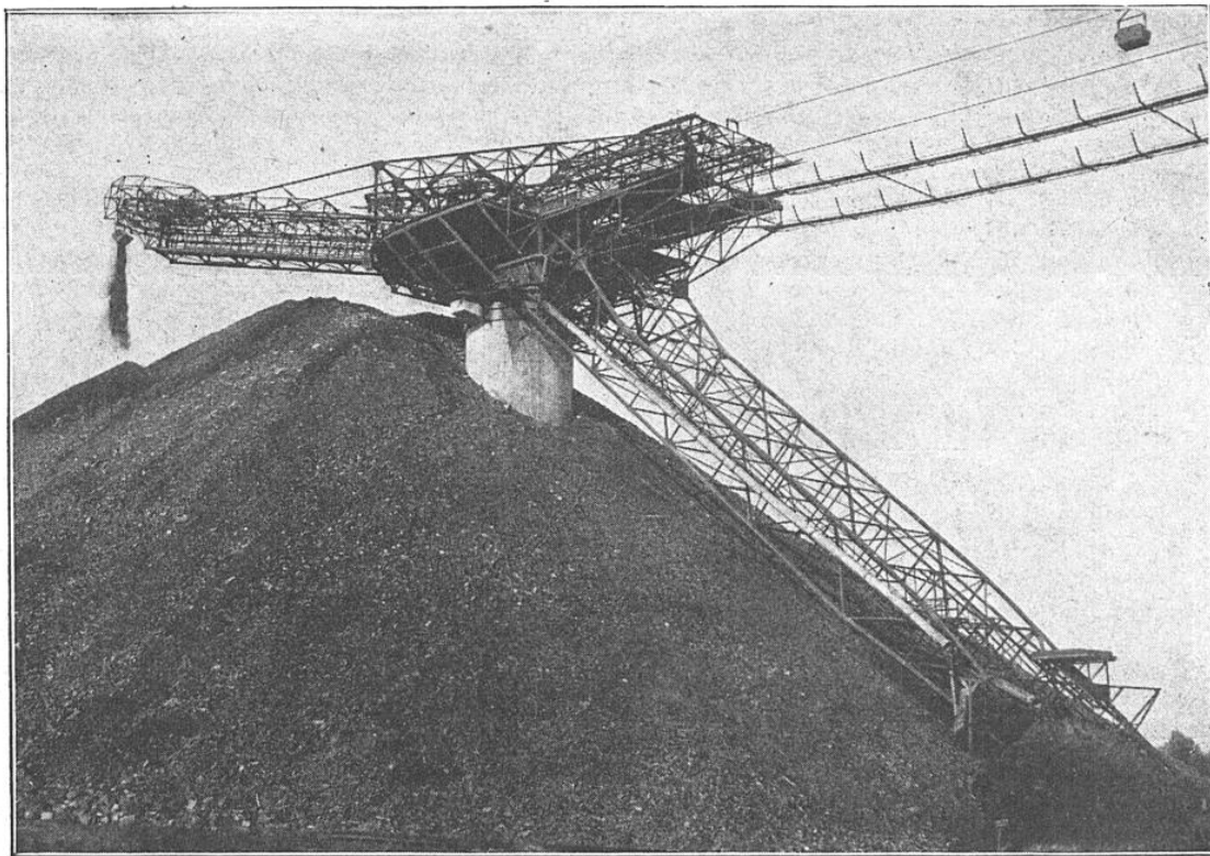
LA STATION DE DÉCHARGEMENT EST ÉRIGÉE SUR UN PILIER EN BÉTON ARMÉ DE 35 MÈTRES DE HAUTEUR
