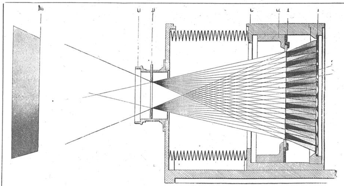
FIG. 4. — COMMENT ON EXÉCUTE UNE PHOTOGRAPHIE « TRAMÉE »
