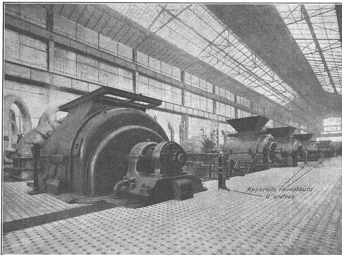
FIG. 6. — LA SALLE DES MACHINES DE GENNEVILLIERS AVEC LES APPAREILS RÉCEPTEURS D'ORDRES MONTÉS SUR PIED A CÔTÉ DES GROUPES GÉNÉRATEURS
