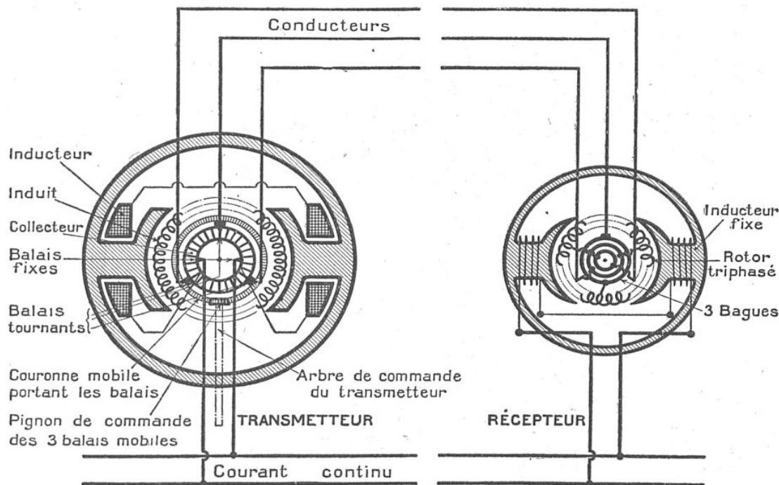
FIG. 2. — SYSTÈME DE TRANSMISSION CONTINUE SAINT-CHAMOND-GRANAT
