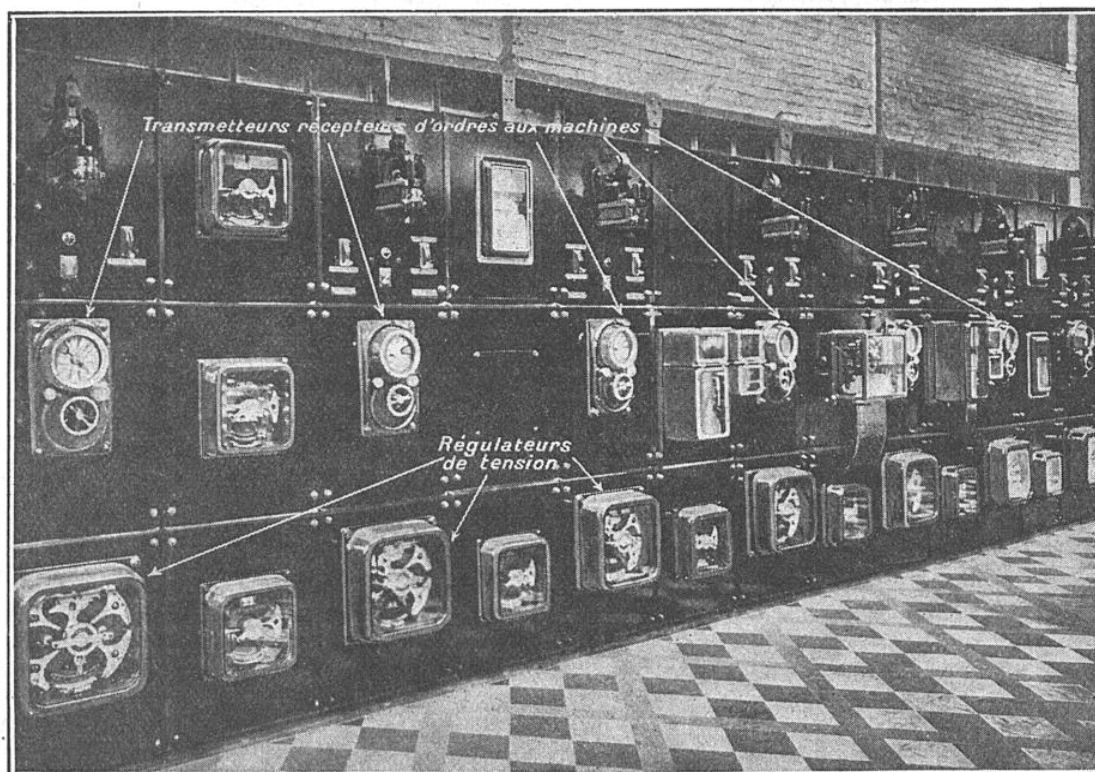
FIG. 5. — AU TABLEAU DE CONTROLE DE LA SUPERCENTRALE DE GENNEVILLIERS SE TROUVENT LES APPAREILS TRANSMETTEURS D'ORDRES EN LIAISON AVEC LA SALLE DES MACHINES
