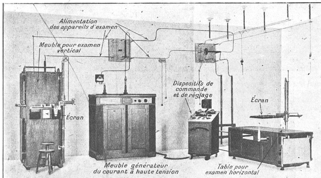
FIG. 9. — VUE D'ENSEMBLE D'UNE INSTALLATION-TYPE DE RADIODIAGNOSTIC
