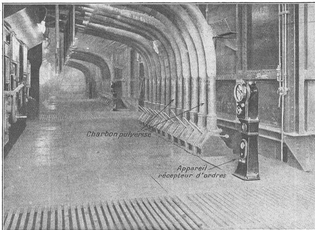
FIG. 7. — LA CHAUFFERIE POSSÈDE AUSSI DES APPAREILS RÉCEPTEURS D'ORDRES
