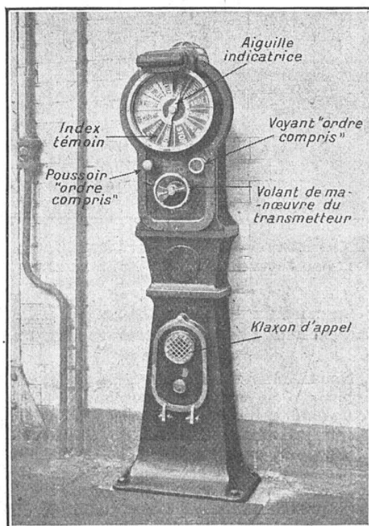
FIG. 3. - POSTE TRANSMETTEUR-RÉCEPTEUR MONTÉ SUR PIED
