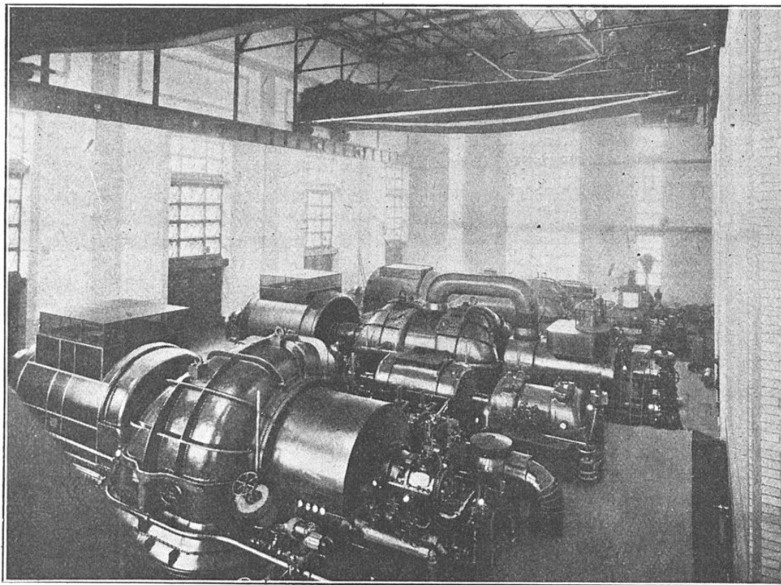
SALLE DES TURBINES DE L'USINE DE LA HUDSON AVENUE, LES UNES SONT DE 50.000 KW, LES AUTRES DE 62.500 KW
