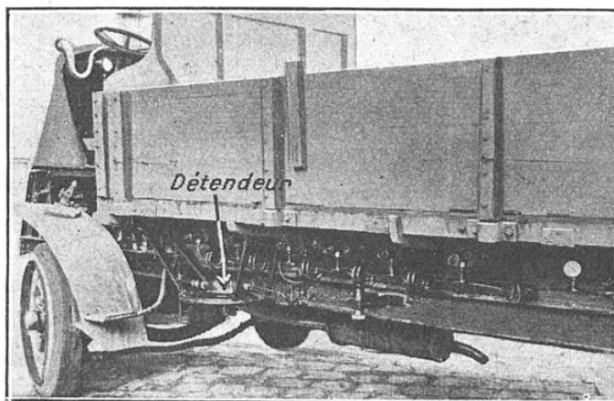
UN CAMION A GAZ ÉQUIPÉ AVEC DES BOUTEILLES D'ACIER Les bouteilles sont rangées transversalement entre la caisse et le châssis. Solution inapplicable à une voiture carrossée pour voyageurs, la place faisant défaut.
