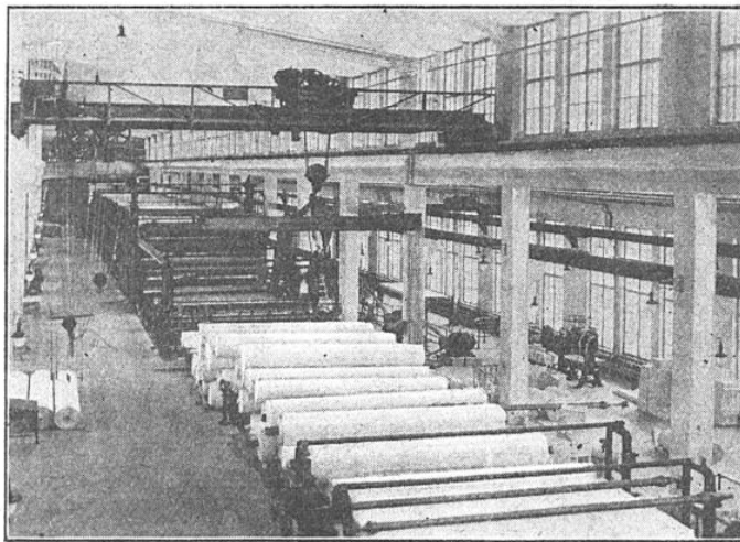
LA PLUS GRANDE MACHINE DE FINLANDE POUR LA FABRICATION DU PAPIER A L'USINE DE VARKAUS
