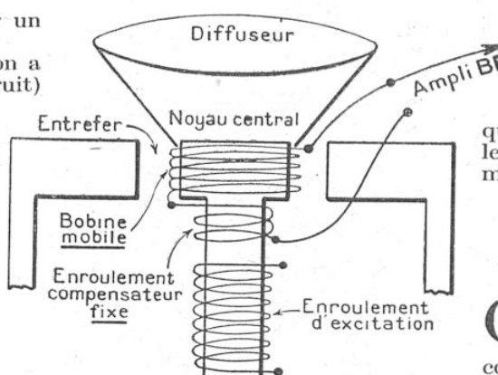
FIG. 3. — COMMENT ON AMÉLIORE UN DIFFUSEUR ÉLECTRODYNAMIQUE AU MOYEN D'UN ENROULEMENT COMPENSATEUR
