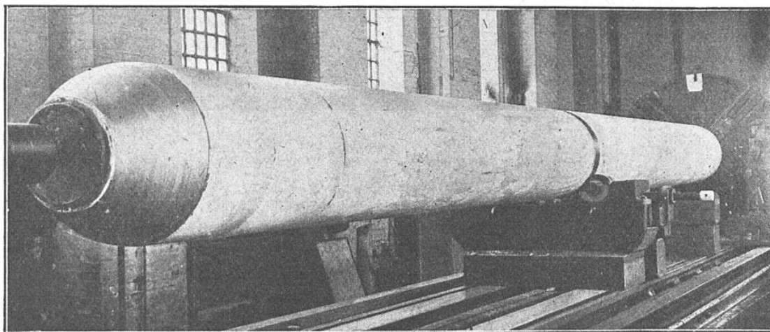
CE CORPS DE CHAUDIÈRE DE LA CENTRALE D'ISSY-LES-MOULINEAUX, DE 10 MÈTRES DE LONG SUR 1 M 20 DE DIAMÈTRE INTÉRIEUR, EST FORMÉ D'UN SEUL BLOC D'ACIER FORGÉ
