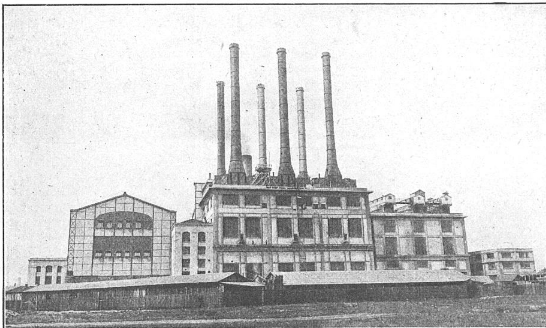
VUE GÉNÉRALE DES EXTENSIONS DE LA CENTRALE THERMO-ÉLECTRIQUE D'ISSY-LES-MOULINEAUX (SEINE) DONT LA PUISSANCE VIENT D'ÊTRE PORTÉE TOUT RÉCEMMENT DE 80.000 A 175.000 KILOWATTS
