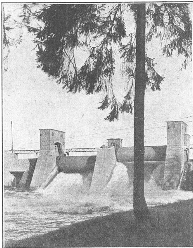
LE BARRAGE D'IMATRA, OU L'ON REMARQUE LES VANNES CYLINDRIQUES PARTICULIÈRES AUX RÉGIONS OU SE PRATIQUE LE FLOTTAGE DU BOIS
