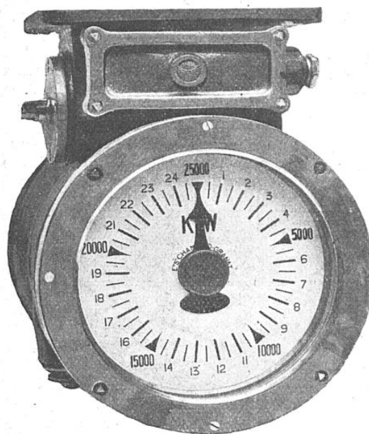
FIG 4. — INDICATEUR CONTINU DE PUISSANCE PERMETTANT DE PROPORTIONNER LA MARCHE DE L'USINE AUX BESOINS DU RÉSEAU
