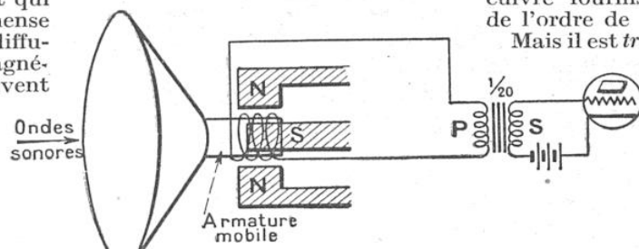
FIG. 2. — MONTAGE D'UN DIFFUSEUR ÉLECTRODYNAMIQUE EN MICROPHONE
