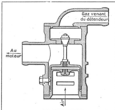
LE MÉLANGEUR QUI TIENT LIEU DE CARBURATEUR DANS LE NOUVEAU SYSTÈME D'ALIMENTATION
