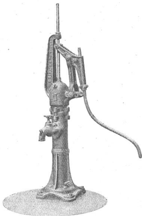
VUE D'ENSEMBLE DE LA POMPE « ROYALE » A GRAND RENDEMENT ET D'UN FONCTION- NEMENT TRÈS DOUX
