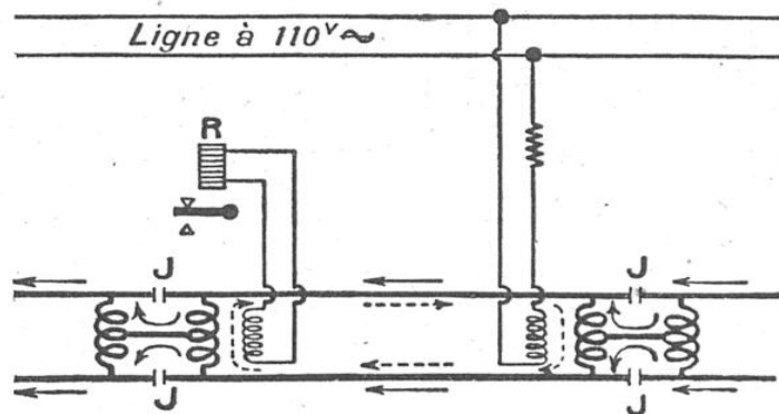
COMMENT EST CONSTITUÉ UN « CIRCUIT DE VOIE » A COURANT ALTERNATIF
