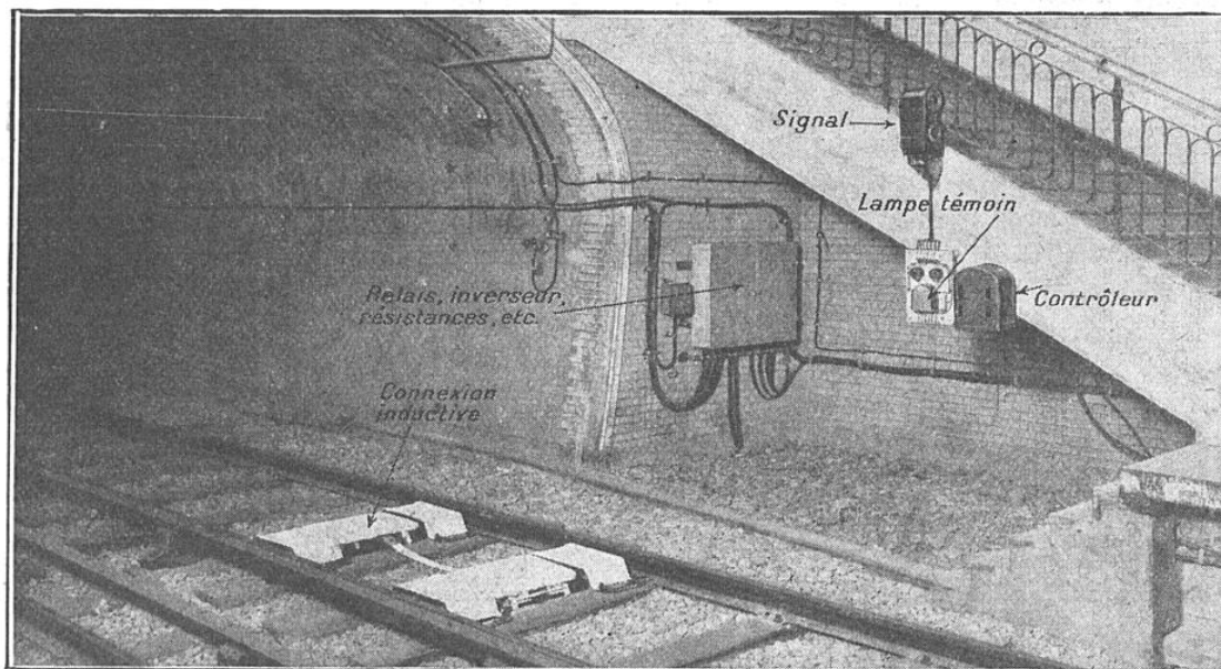
VUE D'UN POSTE DE SIGNALISATION A LA SORTIE D'UNE STATION DU MÉTROPOLITAIN
