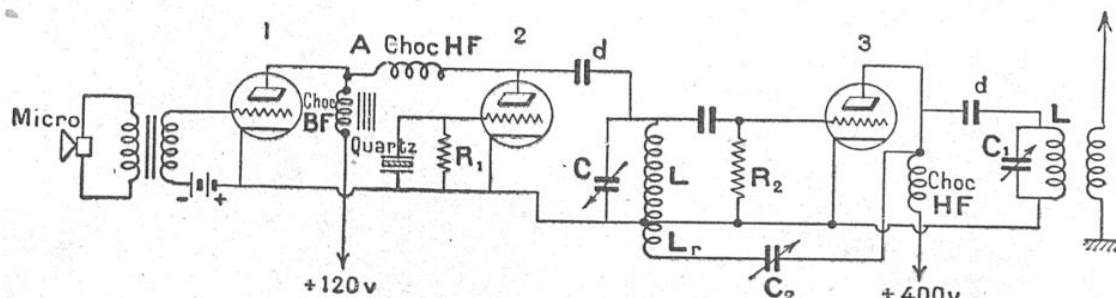
FIG. 4. — SCHÉMA DE MONTAGE D'UN PETIT ÉMETTEUR RADIOPHONIQUE CONTRÔLÉ PAR QUARTZ
