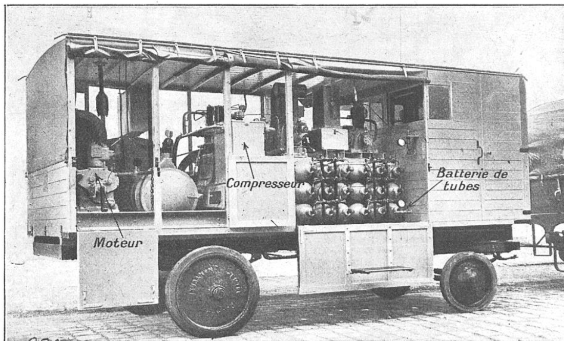
L'USINE DE COMPRESSION AMBULANTE DE L'AUTOMOBILE-CLUB DE FRANCE
