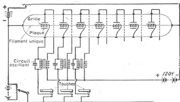
FIG. 2. — UNE LAMPE A PLUSIEURS GRILLES ET PLAQUES, PEUT ÊTRE UTILISÉE POUR L'ORGUE RADIOÉLECTRIQUE
