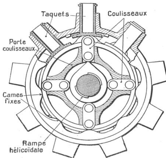
FIG. 2. — SCHÉMA DE COMMANDE DES POMPES A COMBUSTIBLE DU MOTEUR CLERGET
