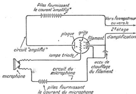
SCHÉMA D'ENSEMBLE DE LA MODULATION DU COURANT AMPLIFIÉ PAR LE COURANT MICROPHONIQUE AVEC L'INTERMÉDIAIRE DE LA LAMPE TRIODE
