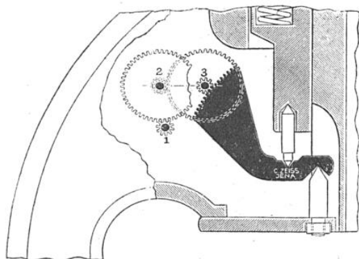
MÉCANISME DU MOUVEMENT LENT D'UN MICROSCOPE ZEISS MODERNE
