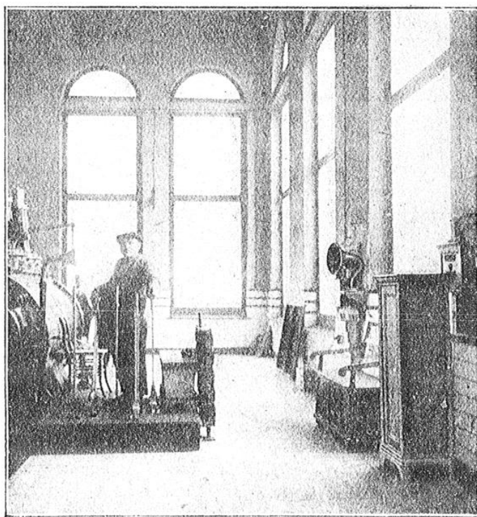
FIG. 1. — PARTIE DE LA SALLE DES MACHINES D'EXTRACTION OU SE TROUVENT, À DROITE, LE RÉCEPTEUR ET LE HAUT-PARLEUR
