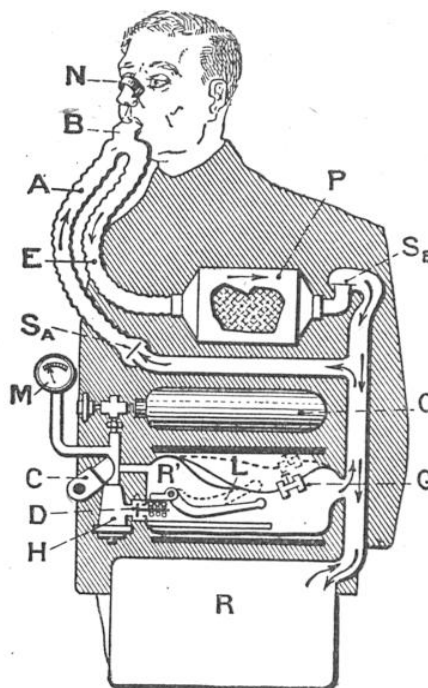
SCHÉMA DE L'APPAREIL « DRÆGER H. S. S. »
