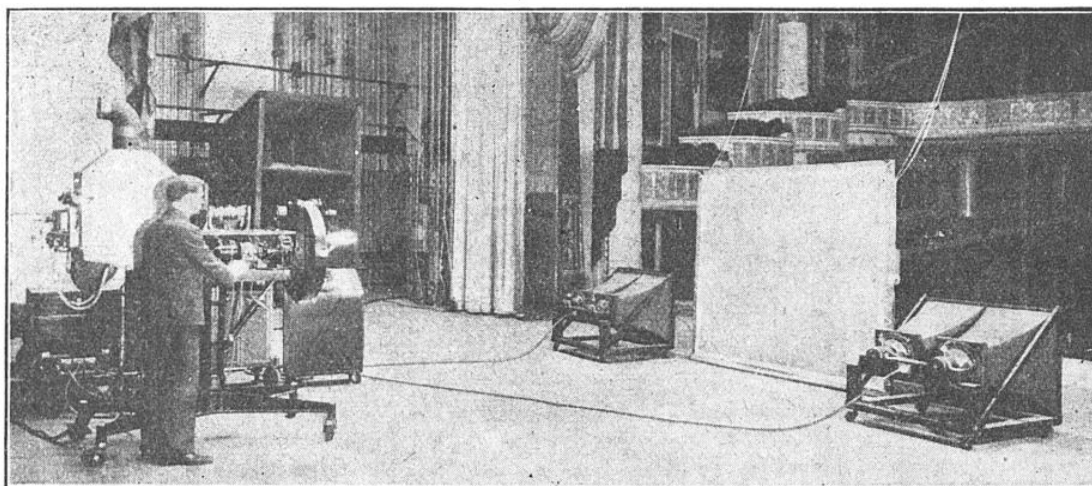
FIG. 1. — INSTALLATION DE SCÈNE POUR LA TÉLÉVISION, A SCHENECTADY (ÉTATS-UNIS) L'appareil de projection est à gauche. L'écran fonctionnant par transparence est sur le devant de la scène du théâtre, flanqué des hauts-parleurs.
