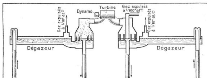
SCHÉMA DE L'INSTALLATION SEMI-INDUSTRIELLE UTILISÉE A OUGRÉE-MARIHAYE (BELGIQUE), PUIS A MATANSAS
