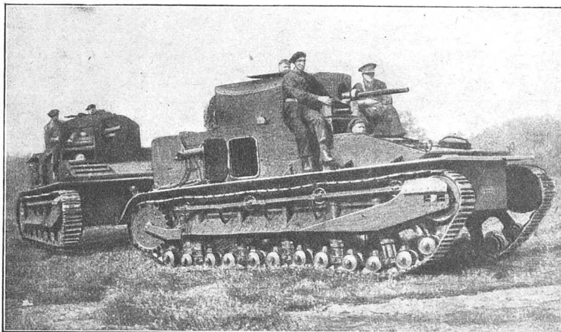
DEUX DES TRENTE TANKS A GRANDE PUISSANCE QUI ONT PRIS PART AUX DERNIÈRES MANŒUVRES ANGLAISES A ALDERSHOT
