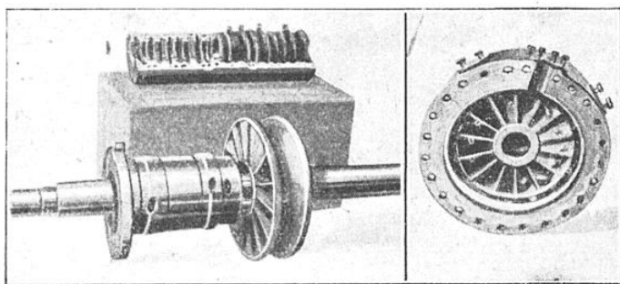
DÉTAILS DU GÉNÉRATEUR DE VAPEUR « FROUDE »
