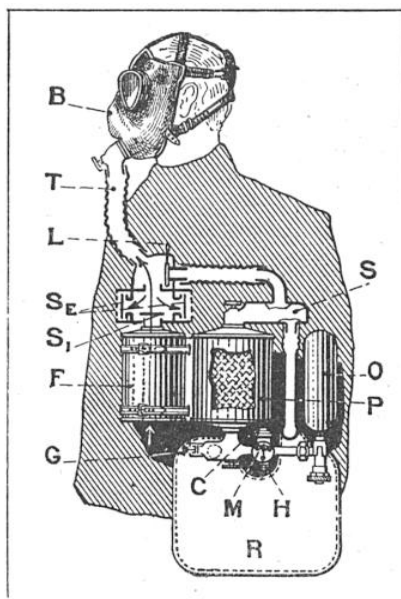
APPAREIL ALLEMAND ULTRA-MODERNE A DOUBLE EFFET
