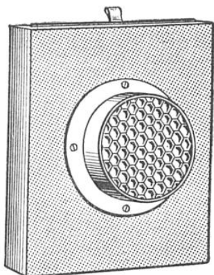
FIG. 3. — ASPECT D'UN CHASSIS POUR PHOTOGRAPHIE INTÉGRALE
