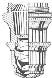
OBJECTIF APO-CHROMATIQUE A IMMERSION (10 LENTILLES)
