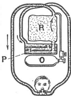
SCHÉMA DE FONCTIONNEMENT DE L'APPAREIL « TISSOT »
