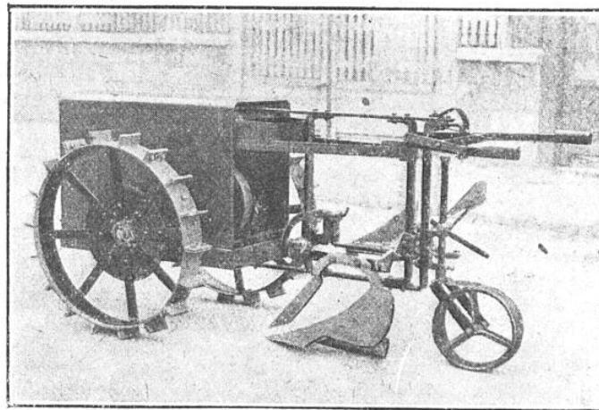
LE TRACTEUR « PÉGASE » PEUT ÊTRE ÉQUIPÉ SOIT AVEC UNE CHARRUE, SOIT AVEC UNE HOUE, SOIT AVEC DES BRISE-MOTTES, ETC.
