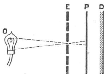
FIG. 4. — DISPOSITIF DE M. ESTANAVE POUR LA VISION DES PHOTOGRAPHIES INTÉGRALES
