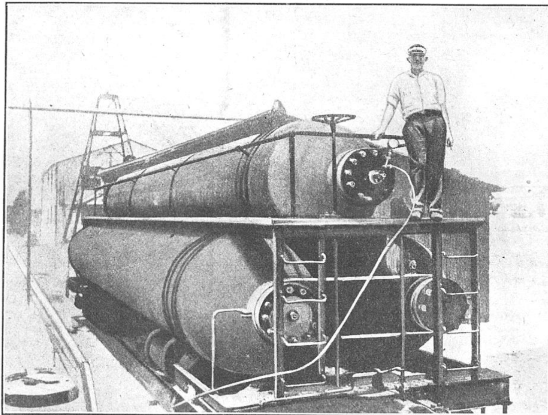
UN DES WAGONS SPÉCIAUX SERVANT AU TRANSPORT DE L'HÉLIUM DEPUIS L'USINE D'AMARILLO (TEXAS) JUSQU'À L'AÉRODROME DE LAKEHURST
