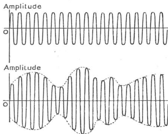
FIG. 7. — MÉCANISME ONDULATOIRE DE LA MODULATION, EN L'ÉTAT ACTUEL DE LA RADIOPHONIE
