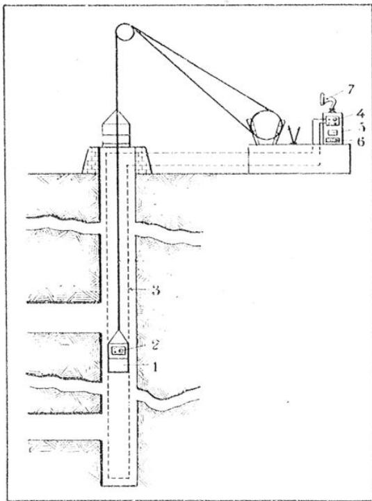
FIG. 2. — SCHÉMA D'INSTALLATION DE SIGNALISATION PAR T. S. F. DANS UNE MINE 1, cage; 2, émetteur; 3, câble de réception; 4, amplificateur-récepteur; 5, 6, accumulateurs; 7, haut-parleur.
