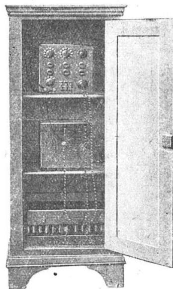
FIG. 5. — L'ARMOIRE RÉCEPTRICE-AMPLIFICATRICE
