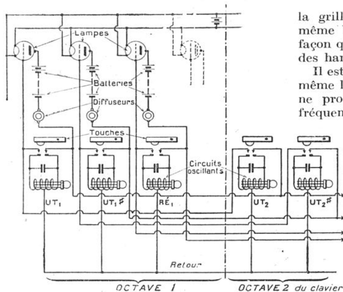
FIG. 1. — SCHÉMA ÉLECTRIQUE DE L'ORGUE RADIO-PHONIQUE MONTRANT LES CIRCUITS OSCILLANTS DES LAMPES CORRESPONDANT A CHAQUE TOUCHE DU CLAVIER
