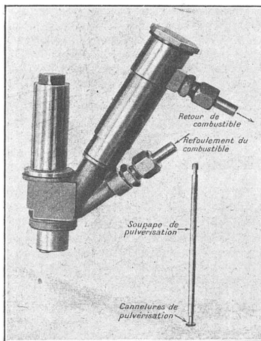
FIG. 5. — ENSEMBLE DU PULVÉRISATEUR D'HUILE A JETS MULTIPLES AVEC, A DROITE, LA SOUPAPE DE PULVÉRISATION
