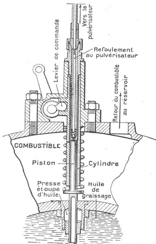
FIG. 1. — DÉTAILS DE LA POMPE A INJECTION D'HUILE LOURDE D'UN CYLINDRE
