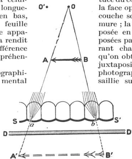
FIG. 1. — PRINCIPE DE LA MÉTHODE PHOTOGRAPHIQUE DE LIPPMANN
