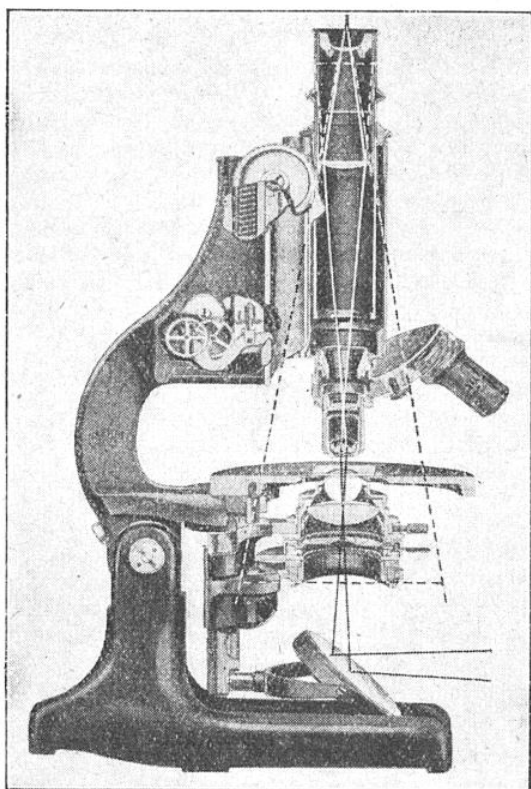
MARCHE DES RAYONS LUMINEUX DANS UN MICROSCOPE
