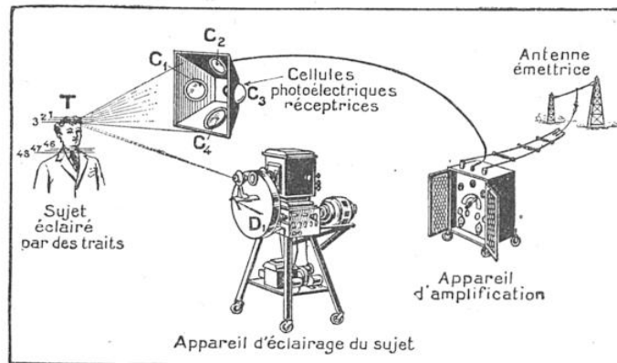
FIG. 3. — MONTAGE DE LA STATION ÉMETTRICE
