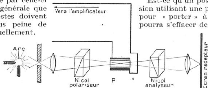
FIG. 5. — COMMENT FONCTIONNE LA CELLULE DE KERR-KAROLUS
