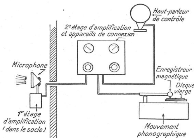
SCHEMA D'ENSEMBLE DE L'ENREGISTREMENT ELECTROMAGNETIQUE DES DISQUES, PLUS COMMUNEMENT APPELE ENREGISTREMENT ELECTRIQUE
