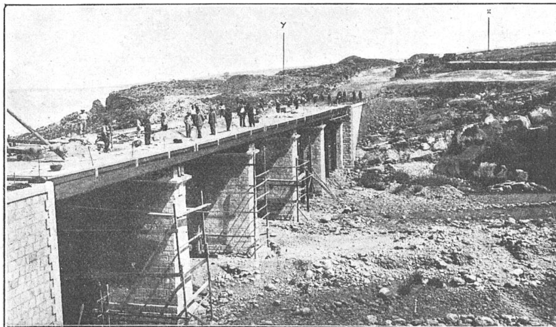
SUR LA COTE MÉDITERRANÉENNE, ENTRE BEYROUTH ET TRIPOLI (LIBAN) Sous l'impulsion des autorités mandataires, les moyens de communication se sont considérablement développés au Levant. Pont en béton armé, construit pour raccourcir la route. X, ancienne route ;
