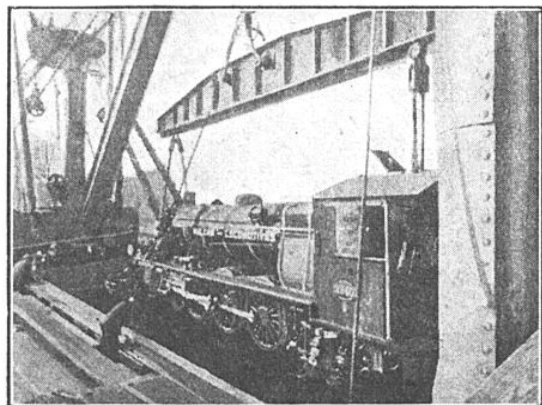
LA LOCOMOTIVE EST DESCENDUE DIRECTEMENT DANS LA CALE
