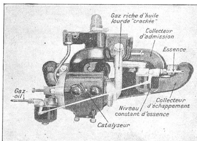
FIG. 1. — VUE D'ENSEMBLE DU CARBURATEUR CHIMIQUE « CATALEX » QUI PERMET L'EMPLOI DES HUILES LOURDES SUR LES MOTEURS ORDINAIRES A EXPLOSIONS A ESSENCE
