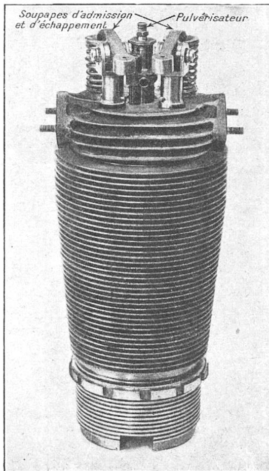
FIG. 4. — UN DES CYLINDRES DU MOTEUR CLERGET 100 CHEVAUX AVEC LES SOUPAPES ET LE PULVÉRISATEUR DE COMBUSTIBLE
