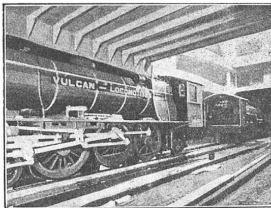
A FOND DE CALE, LES LOCOMOTIVES REPOSENT SUR LES RAILS ET SONT SOIGNEUSEMENT ARRIMÉES
