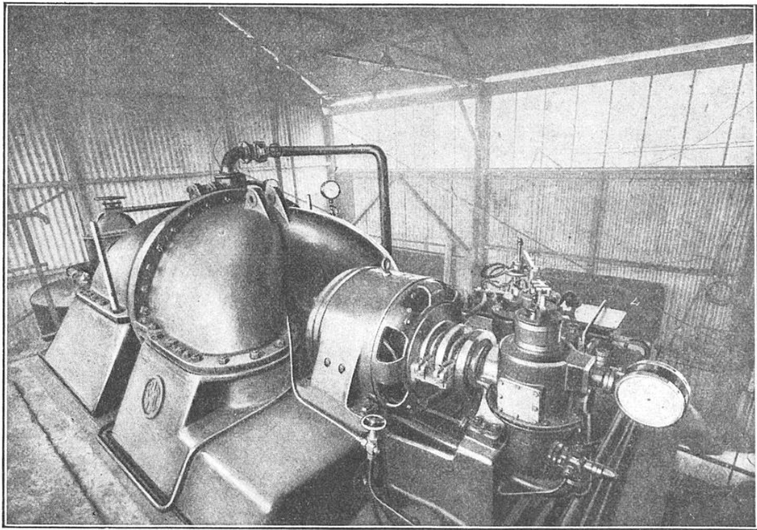
LE GROUPE TURBO-GÉNÉRATEUR DE 50 KILOWATTS A L'USINE D'ESSAIS DE MATANSAS
