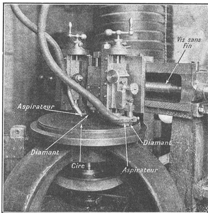
LE POLISSAGE AU TOUR AVEC UNE POINTE DE DIAMANT DE LA SURFACE DE CIRE D'UN DISQUE VIERGE, AVANT L'ENREGISTREMENT (USINE COLUMBIA)
