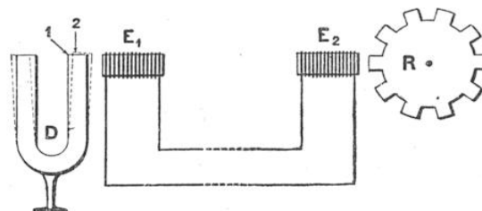
FIG. 8. — PRINCIPE DE LA SYNCHRONISATION PAR « ROUE PHONIQUE »
