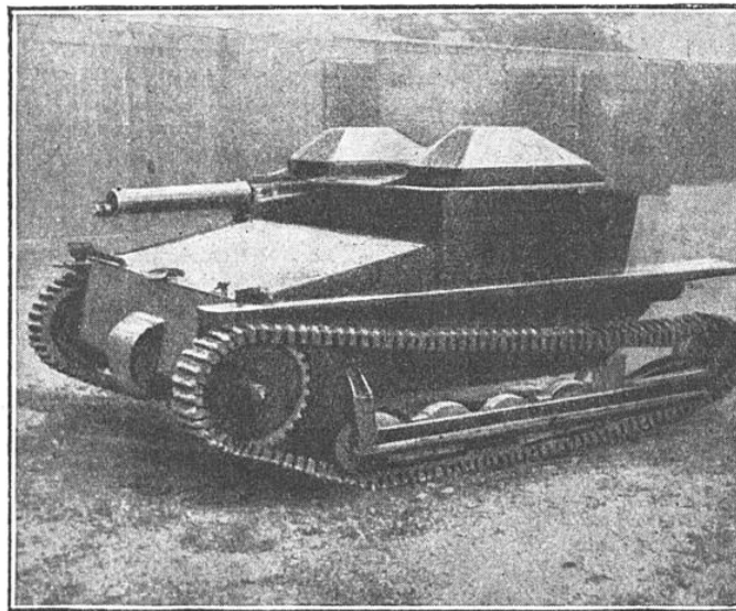
VUE D'ENSEMBLE DU LÉGER CHAR BLINDÉ « CARDEN LOYD », DONT LE TOIT A ÉTÉ MUNI D'UN BLINDAGE SPÉCIAL POUR LE PROTÉGER, PENDANT LES COMBATS DE VILLE, DES COUPS PROVENANT DES ÉTAGES SUPÉRIEURS
