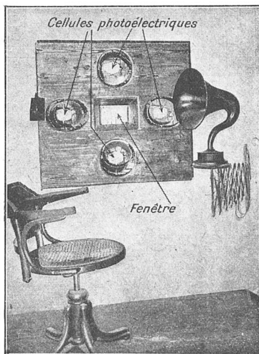
FIG. 9. — LE PANNEAU DES CELLULES PHOTO-ÉLECTRIQUES AU POSTE DE TRANSMISSION DE L'APPAREIL BARTHÉLÉMY
