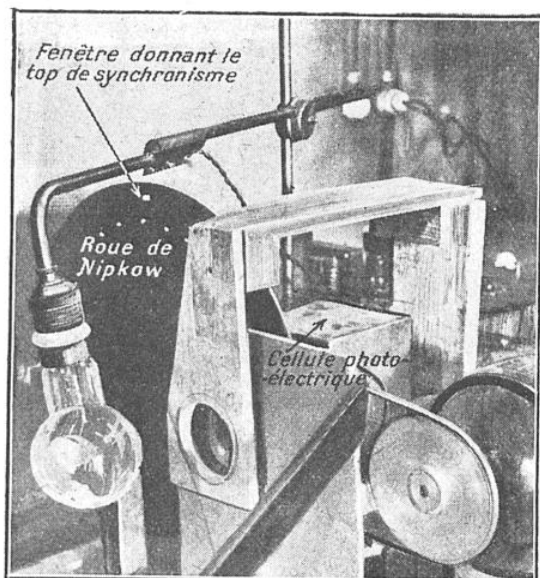
FIG. 11. — DISPOSITIF D'EXPÉRIENCE MONTRANT LE PRINCIPE DE LA TRANSMISSION DU SYNCHRONISME, DANS LE PROCÉDÉ DE TÉLÉVISION BARTHÉLÉMY
