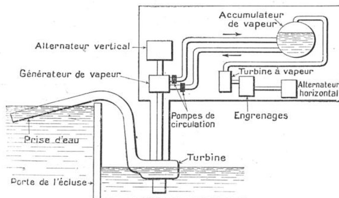
SCHEMA GÉNÉRAL DE L'USINE EXPÉRIMENTALE INSTALLÉE EN ANGLETERRE, AU PORT D'AVONMOUTH
