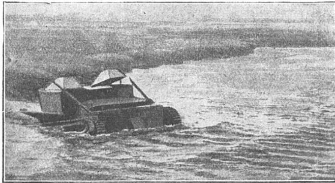
LE LÉGER CHAR BLINDÉ « CARDEN LOYD » PEUT TRAVERSER UNE RIVIÈRE, SI L'EAU N'EST PAS TROP PROFONDE. On remarque sur le char un des panneaux blindés soulevé.
