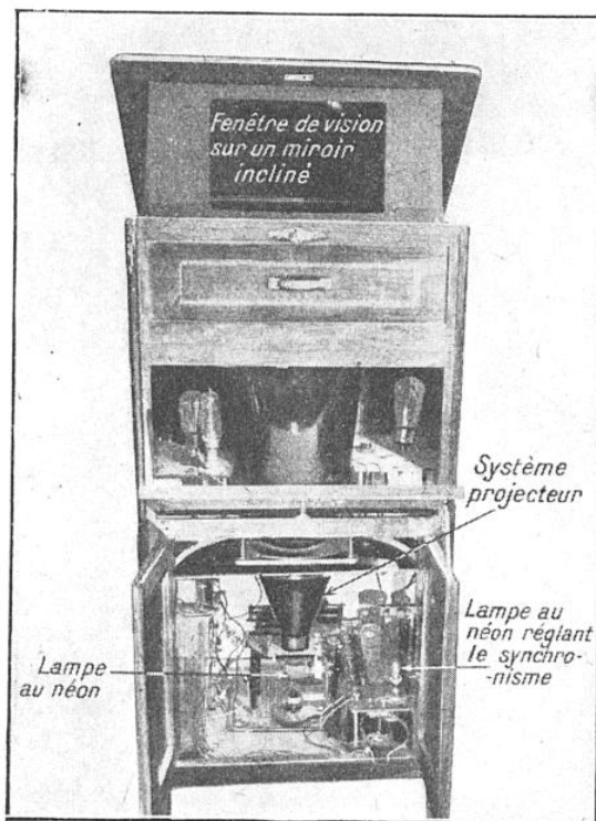
FIG. 12. — LE POSTE RÉCEPTEUR DE TÉLÉVISION BARTHÉLÉMY
