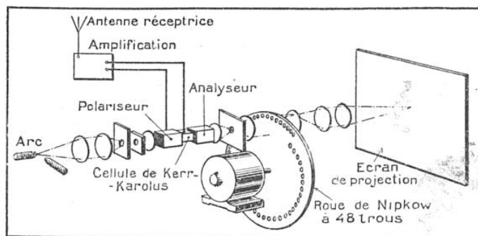
FIG. 6. — DÉTAIL DE L'APPAREIL RÉCEPTEUR
