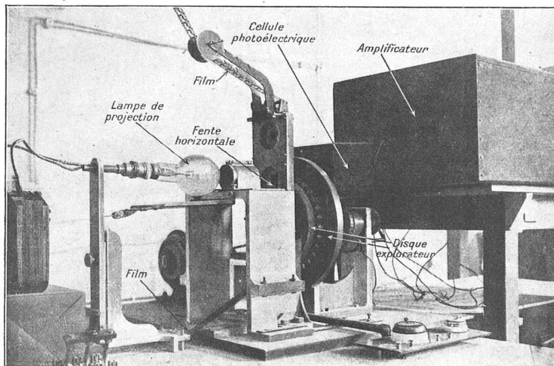
FIG. 13. — LE TÉLÉCINÉMA BARTHÉLÉMY : POSTE DE TRANSMISSION.
