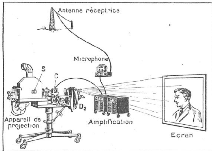
FIG. 4. — MONTAGE DE LA STATION RÉCEPTRICE
