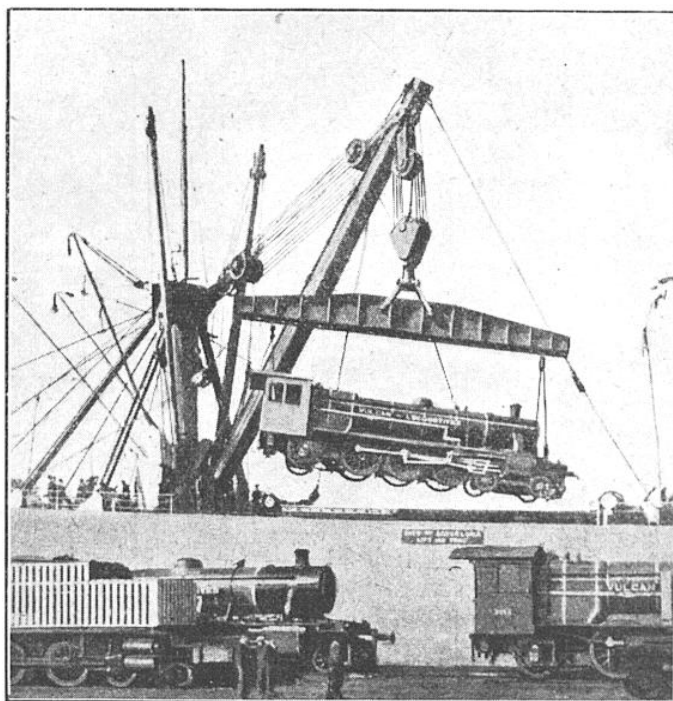
UNE LOCOMOTIVE DE 75 TONNES EST CHARGÉE A BORD DU CARGO ANGLAIS « CITY-OF-BARCELONA »
