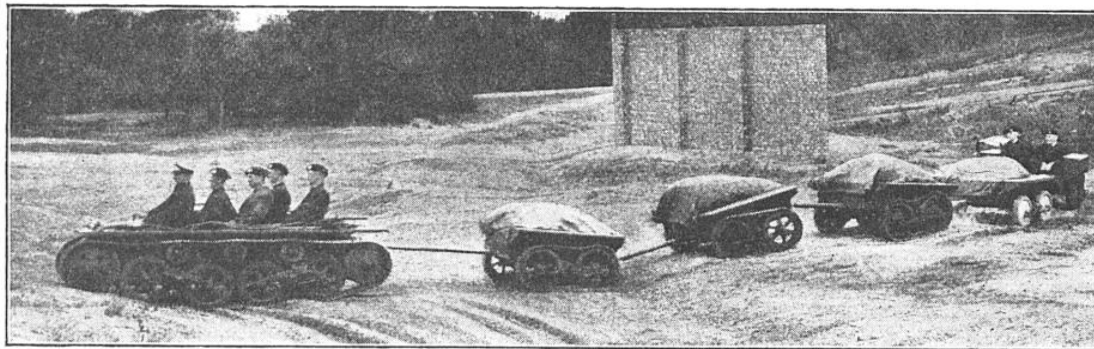
LES TRACTEURS A CHENILLES ANGLAIS REMPLACENT LES CHEVAUX POUR ASSURER LE TRANSPORT DU MATÉRIEL ET LE RAVITAILLEMENT EN MUNITIONS
