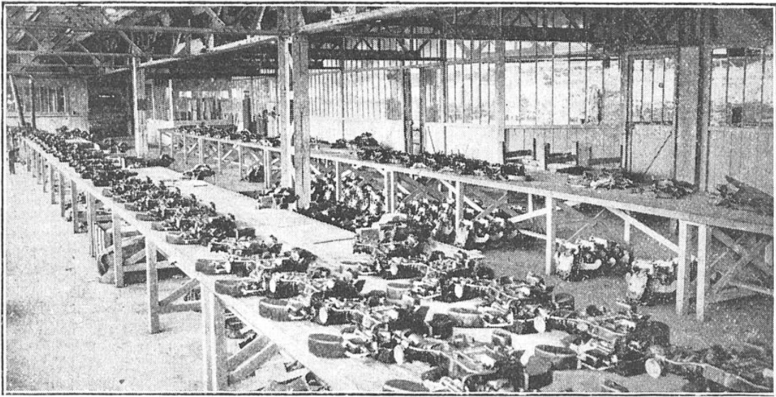
FIG. 2. — UNE CHAÎNE DE MONTAGE DU CARBURATEUR CHIMIQUE PENDANT SA FABRICATION
