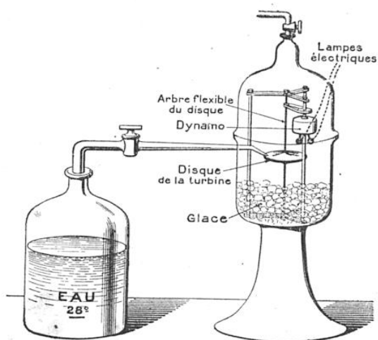
SCHÉMA DE L'EXPÉRIENCE RÉALISÉE EN 1926, A L'ACADÉMIE DES SCIENCES
