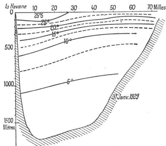
RÉSULTAT DE SONDAGES OPÉRÉS PAR M. IDRAC ENTRE LA HAVANE ET LA POINTE SUD-EST DE LA FLORIDE, EN VUE DE DÉTERMINER LA VARIATION DE LA TEMPÉRATURE DE LA SURFACE AU FOND
