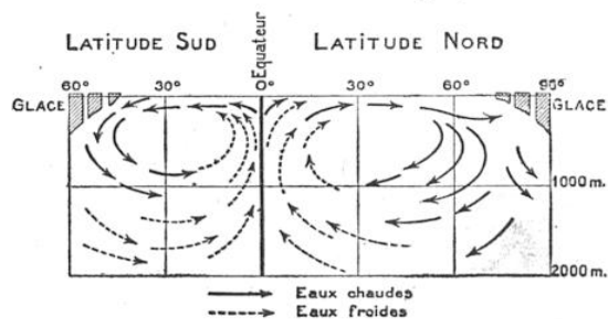
SCHÉMA DE LA CIRCULATION GÉNÉRALE DES EAUX FROIDES PROFONDES ET DES EAUX CHAUDES DE SURFACE DANS LES OCÉANS
