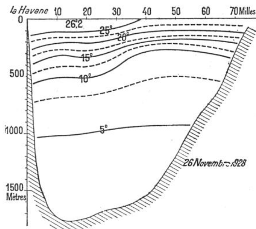
RÉSULTAT DE SONDAGES OPÉRÉS PAR M. IDRAC ENTRE LA HAVANE ET LA POINTE SUD-EST DE LA FLORIDE, EN VUE DE DÉTERMINER LA VARIATION DE LA TEMPÉRATURE DE LA SURFACE AU FOND
