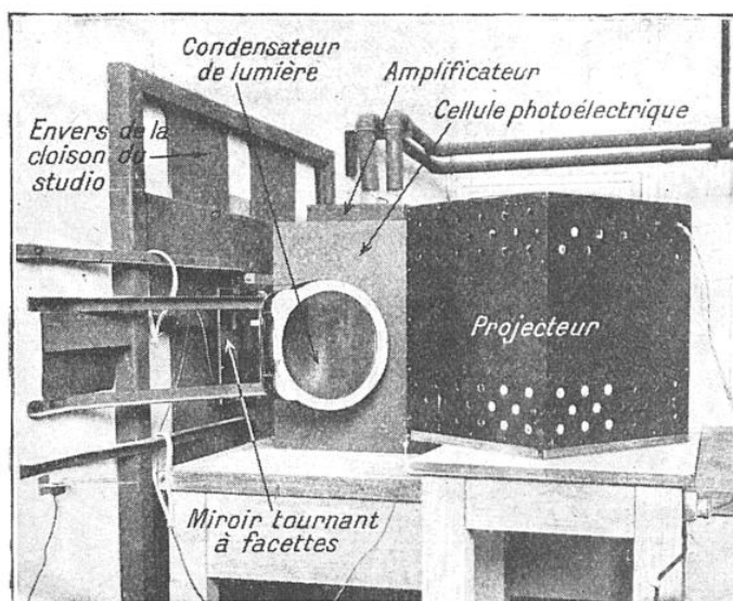
FIG. 10. — L'ENVERS DU PANNEAU PRÉCÉDENT (POSTE DE TRANSMISSION)
