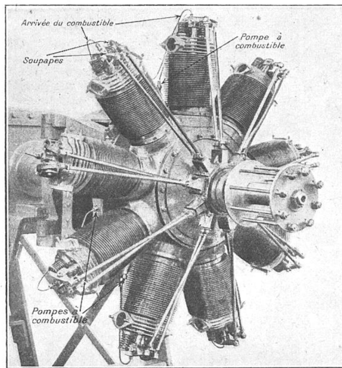
FIG. 3. — ENSEMBLE DU MOTEUR CLERGET, A HUILE LOURDE, DE 100 CHEVAUX
