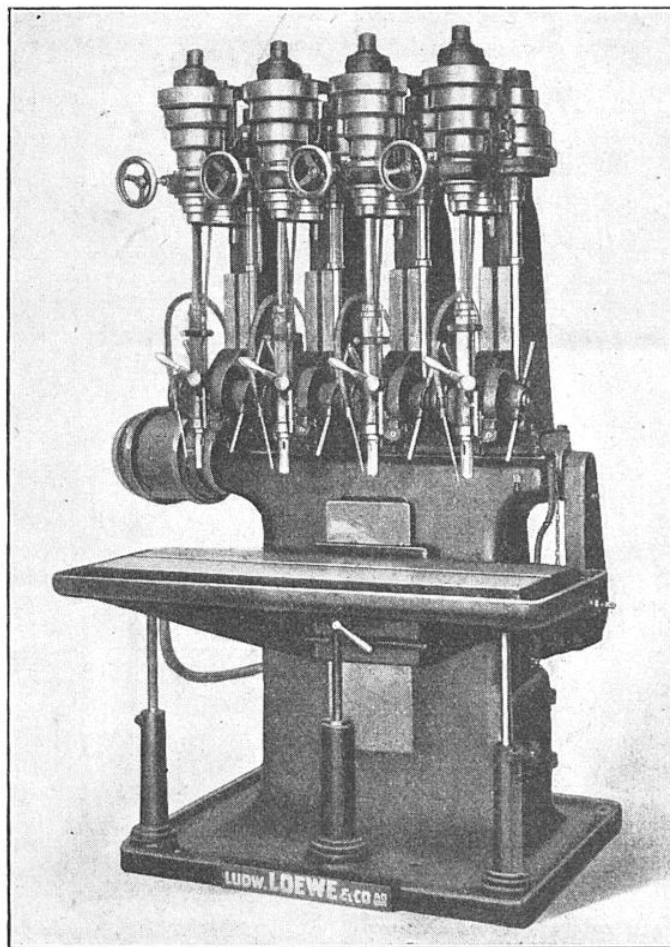
FIG. 1. — PERCEUSE AUTOMATIQUE A QUATRE BROCHES, A GRAND RENDEMENT, POUVANT ÊTRE ALIMENTÉE PAR UN SEUL OUVRIER
