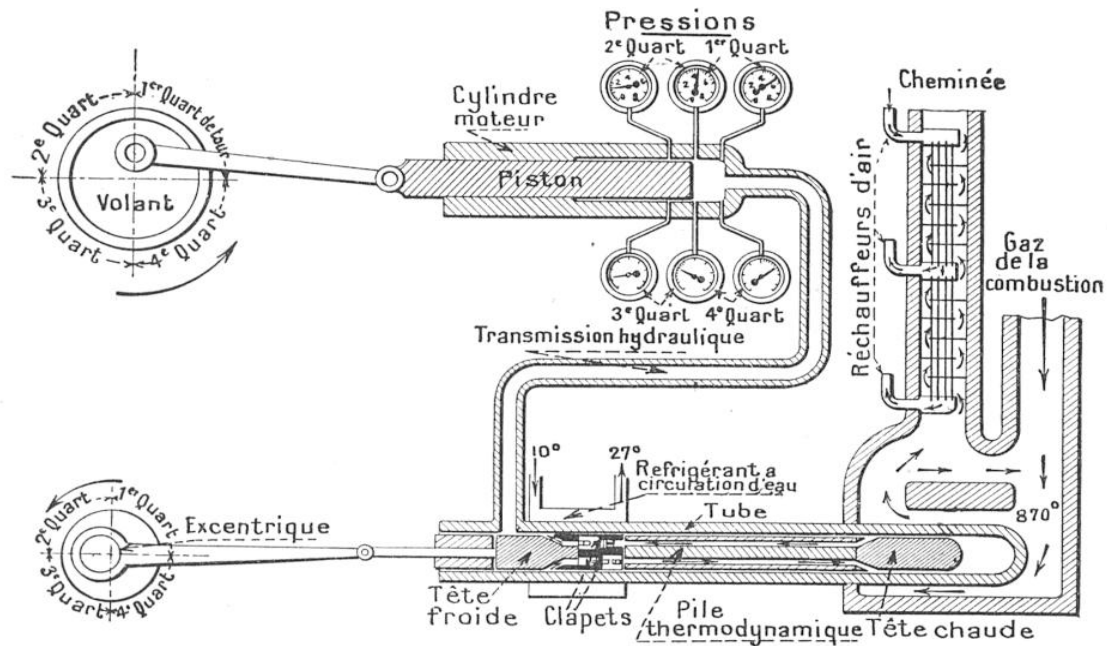
FIG. 1. — SCHÉMA MONTRANT LA DISPOSITION DES ORGANES ET LE FONCTIONNEMENT DU MOTEUR THERMIQUE MALONE, UTILISANT LA DILATATION DE L'EAU LIQUIDE
