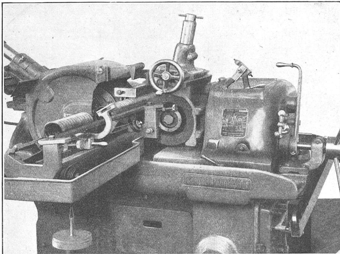
FIG. 6. — MACHINE AUTOMATIQUE POUR LA RECTIFICATION « A L'ENFILADE » DE PIÈCES CYLINDRIQUES, DE BAGUES PAR EXEMPLE, QUI CIRCULENT ENTRE DES MEULES
