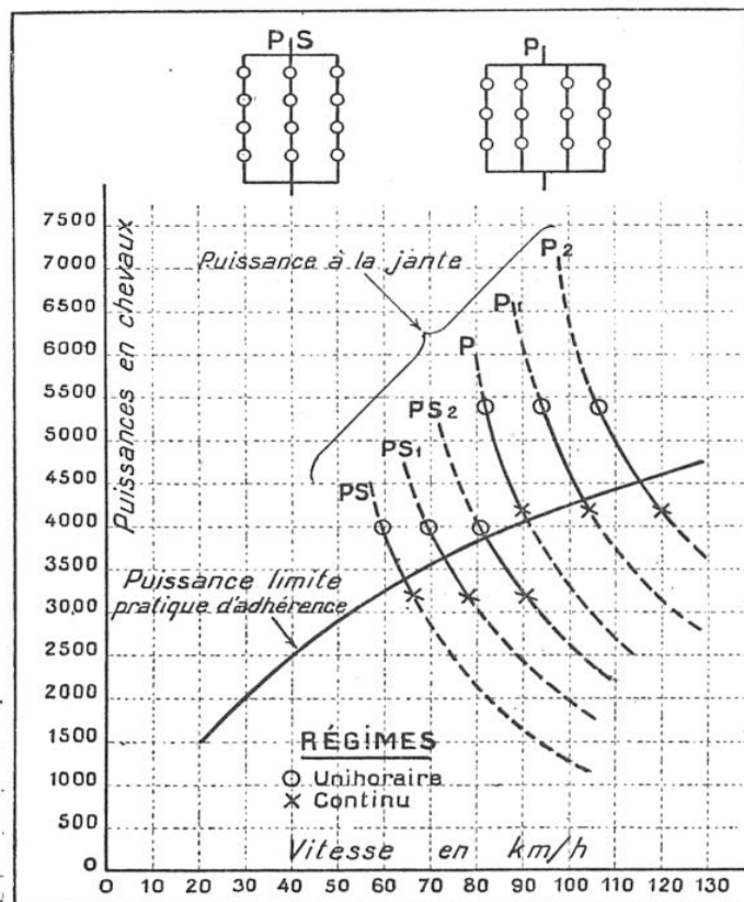
FIG. 4. — VARIATION DE LA PUISSANCE A LA JANTE DE LA LOCOMOTIVE ÉLECTRIQUE DE 6.000 CH DU P.-L.-M.
