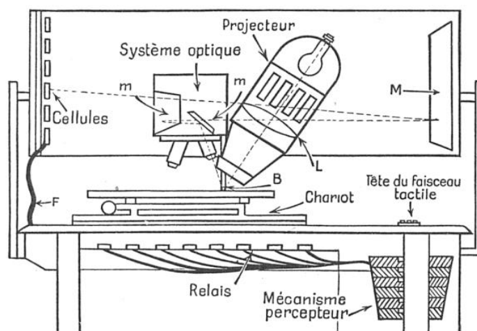
SCHÉMA DE FONCTIONNEMENT DU PHOTOÉLECTROGRAPHE
