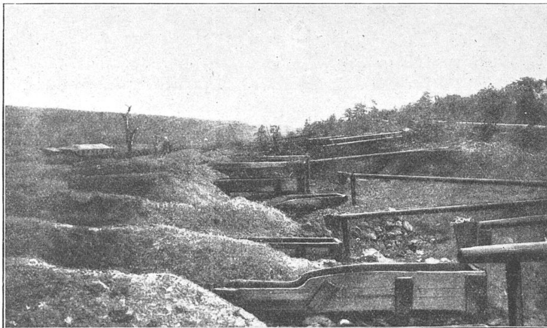
BATTERIE DE « SLUICES », DANS UNE MINE D'ÉTAÏN, AU CONGO BELGE
