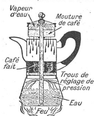
COUPE DE LA CAFETIÈRE MONTRANT LA CIRCULATION DE L'EAU ET DU CAFÉ
