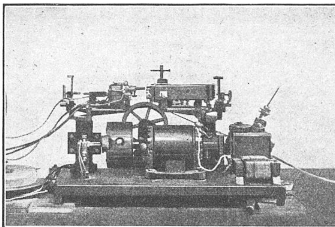
FIG. 4. — CHRONOGAPHE ABRAHAM DE L'OBSERVATOIRE DE ZI KA WEÏ (CHINE), SERVANT A L'ENREGISTREMENT DES SIGNAUX HORAIRES DE T. S. F.
