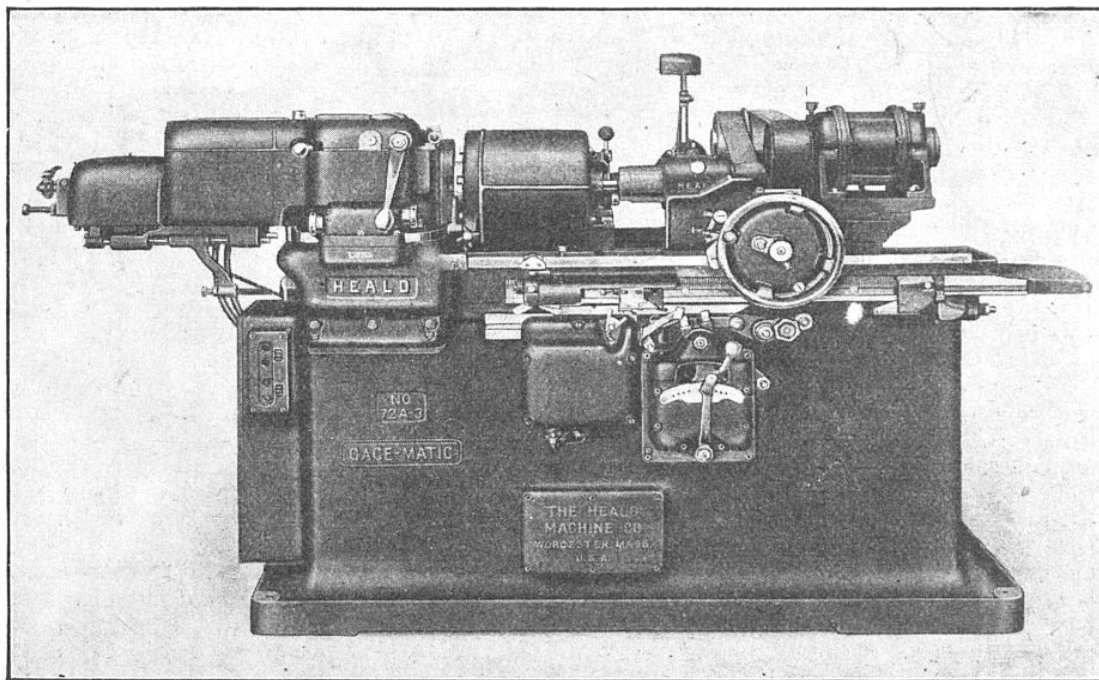
FIG. 9. — MACHINE AUTOMATIQUE A RECTIFIER INTÉRIEUREMENT, POUVANT VÉRIFIER ELLE-MÊME LE DEGRÉ DE PRÉCISION DE SON TRAVAIL. (VOIR FIG. 10)
