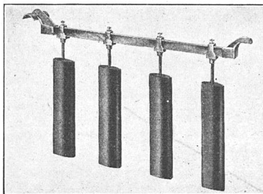
FIG. 5. — ANODES SOLUBLES EN NICKEL, SUSPENDUES A DES CROCHETS EN MÉTAL INOXYDABLE, UTILISÉES POUR LE NICKELAGE ÉLECTROLYTIQUE DE L'ALUMINIUM
