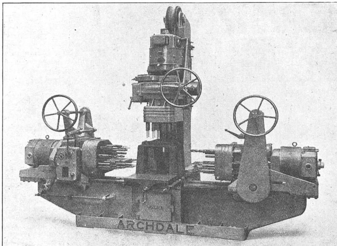
FIG. 2. — PERCEUSE A TROIS TÊTES ET A SOIXANTE-DIX-SEPT BROCHES, POUR L'USINAGE EN GRANDE SÉRIE DES BLOCS-CYLINDRES DE MOTEURS D'AUTOMOBILES
