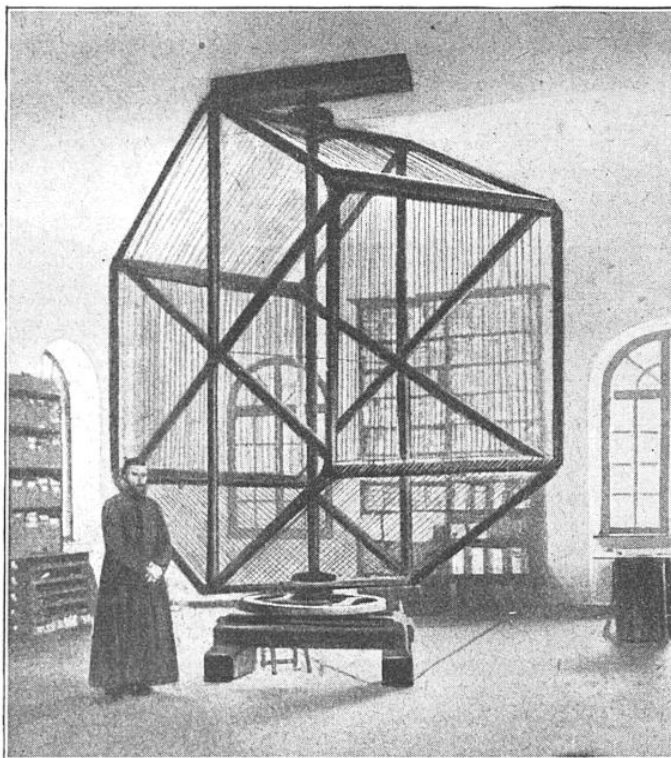
FIG. 5. — LE COLLECTEUR D'ONDES, POUR LA RÉCEPTION DES SIGNAUX HORAIRES DE TÉLÉGRAPHIE SANS FIL, À L'OBSERVATOIRE DE ZI KA WEÏ (CHINE)
