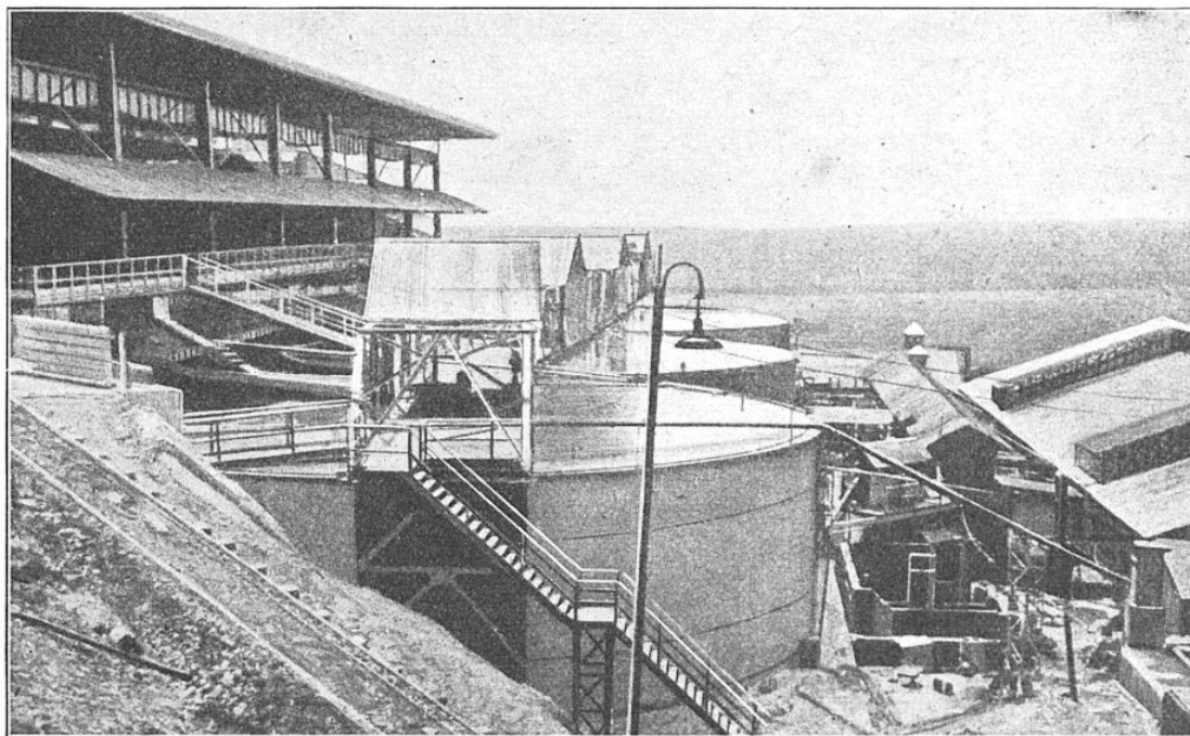
TANKS POUR L'ENRICHISSEMENT DU MINERAI DE CUIVRE PAR LE PROCÉDÉ DE FLOTTAGE (EN PRÉSENCE D'UNE ÉMULSION D'HUILE), AUX USINES DE PANDA, DANS LE HAUT-KATANGA
