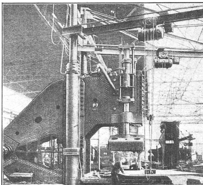
CETTE PRESSE HYDRAULIQUE, HAUTE DE 14 MÈTRES, A ÉTÉ UTILISÉE POUR LE CINTRAGE DES TOLES DU NOUVEAU CUIRASSÉ ALLEMAND « DEUTSCHLAND »
