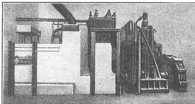
FIG. 3. — LE SECOND MOTEUR INDUSTRIEL MALONE, CAPABLE DE DÉVELOPPER UNE PUISSANCE DE 100 CH A gauche, le foyer soigneusement calorifugé dans lequel baignent les têtes de vingt piles thermodynamiques. Ces piles actionnent deux cylindres. Le rendement indiqué a été de 27 pour cent. Cette machine fonctionne, non avec de l'eau, mais avec du mercure.
