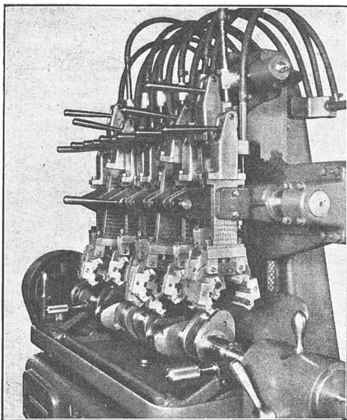
FIG. 7. — MACHINE AUTOMATIQUE SPÉCIALE POUR LA RECTIFICATION DES PORTÉES DES VILEBREQUINS D'AUTOMOBILES
