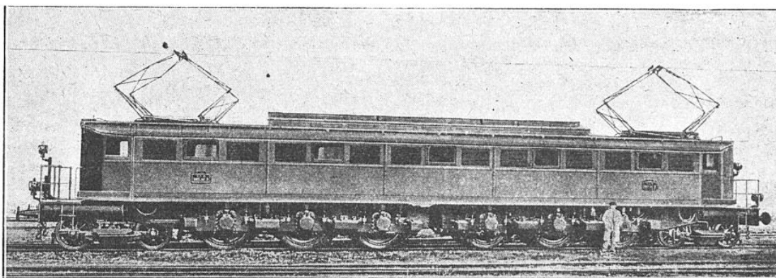
FIG. 8. — LOCOMOTIVE ÉLECTRIQUE DE 6.000 CH, DU P.-L.-M.
