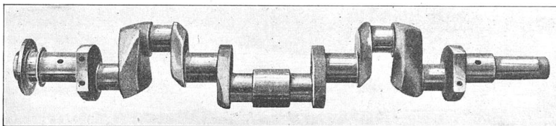
FIG. 4. — VILEBREQUIN DE MOTEUR A EXPLOSIONS, DONT LES PARTIES FROTTANTES, PORTÉES (REPOSANT SUR LES PALIERS) ET SOIES (TOURNANT DANS LES TÊTES DE BIELLES), ONT ÉTÉ SOUMISES A LA NITRURATION POUR EN RÉDUIRE L'USURE
