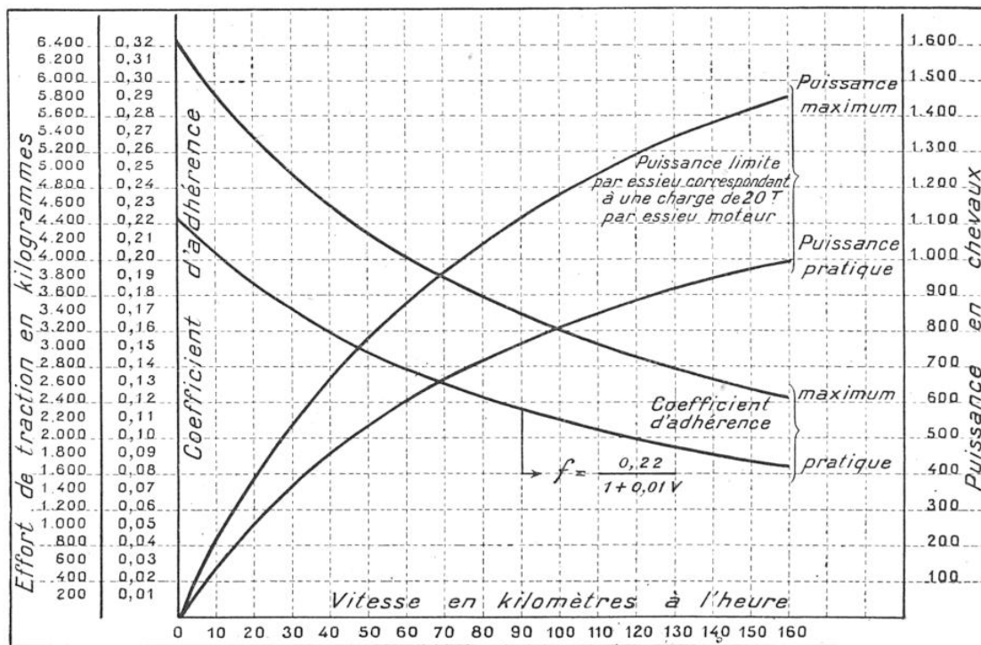
FIG. 1. — COURBES MONTRANT COMMENT VARIENT, AVEC LA VITESSE, LE COEFFICIENT D'ADHÉRENCE ET LA PUISSANCE QUE L'ON PEUT DÉVELOPPER À LA JANTE D'UN ESSIEU MOTEUR PORTANT UNE CHARGE DE 20 TONNES
