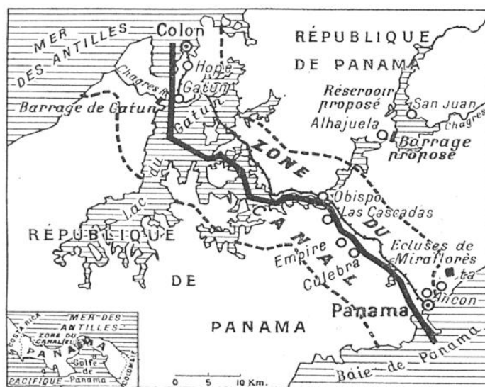
LE CANAL DE PANAMA ET L'EMPLACEMENT DU BARRAGE PROJETÉ D'ALHAJUELA
