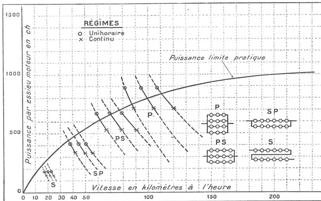
FIG. 2. — COURBES CARACTÉRISTIQUES DE FONCTIONNEMENT DE LA LOCOMOTIVE ÉLECTRIQUE DE 6.000 CH DU RÉSEAU P.-L.-M.
