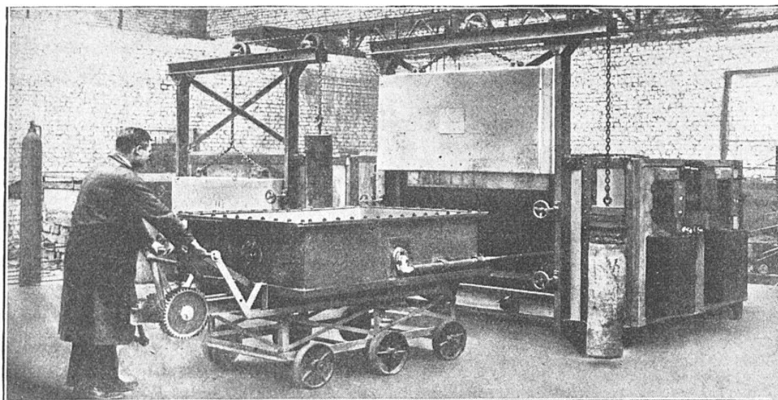
FIG. 1. — FOUR CHAUFFÉ ÉLECTRIQUEMENT POUR LA NITRURATION DE L'ACIER Les pièces à nitrurer sont placées dans la cuve en acier que l'on va introduire dans le four.
