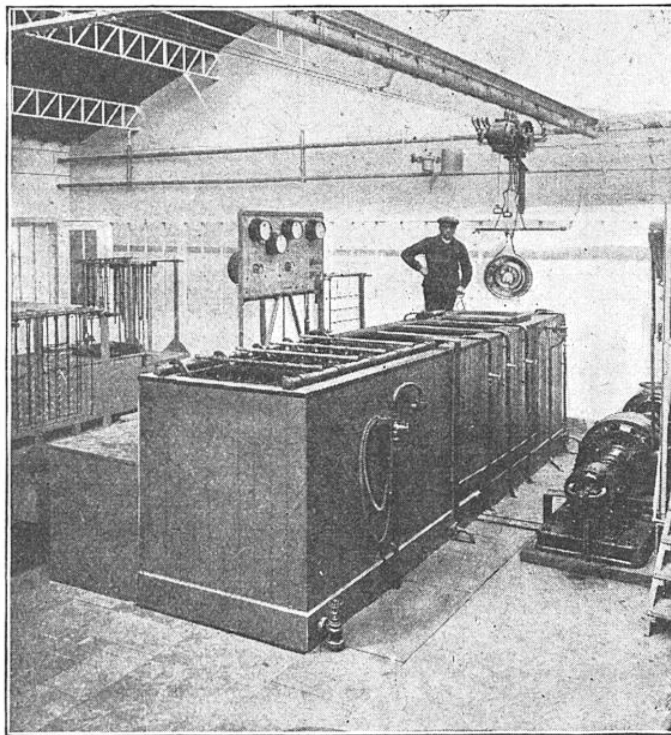
FIG. 6. — ENSEMBLE D'UN DISPOSITIF D'ÉLECTROLYSE POUR LE CHROMAGE DE L'ALUMINIUM
