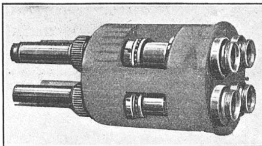
FIG. 4. — TAMBOUR A QUATRE BROCHES POUR TOUR MULTIBROCHES
