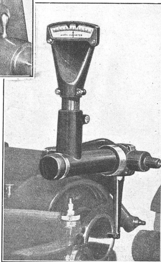
FIG. 8. — LE MINIMÈTRE DE HIRTH, MONTÉ ICI POUR LE CONTRÔLE DES ALÉSAGES, PERMET DE SE RENDRE COMPTE, PAR LECTURE DIRECTE, DU DEGRÉ DE PRÉCISION OBTENU DANS LA RECTIFICATION D'UNE PIÈCE
