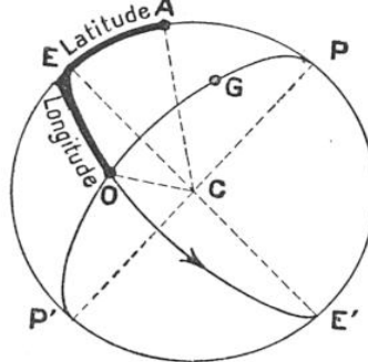
FIG. 1. — COMMENT ON DÉFINIT LA LONGITUDE ET LA LATITUDE D'UN POINT A LA SURFACE DE LA TERRE P-P' étant la ligne des pôles, la longitude de A est mesurée par l'angle du méridien P-A-P' avec le méridien origine P-O-P' passant par Greenwich (G). La latitude est mesurée par l'angle de A-C avec le plan de l'équateur E-E'.
