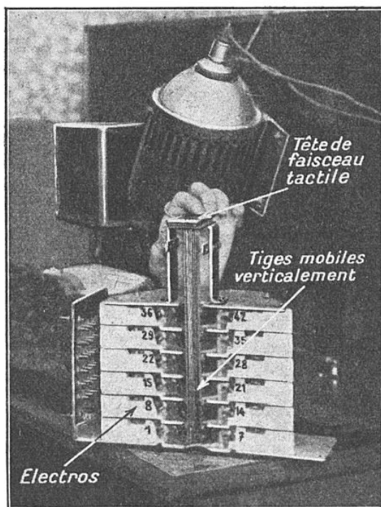
LE « RÉCEPTEUR » DU PHOTOÉLECTROGRAPHE Quarante-deux électros (correspondant aux quarante-deux cellules photoélectriques) sont groupés en demi-cercle autour du faisceau tactile, dont ils repoussent les quarante-deux tiges verticales dans l'ordre qu'indique l'ombre portée de la lettre sur l'échiquier des cellules. Ce curieux sélecteur est l'invention personnelle de Mme Thomas.
