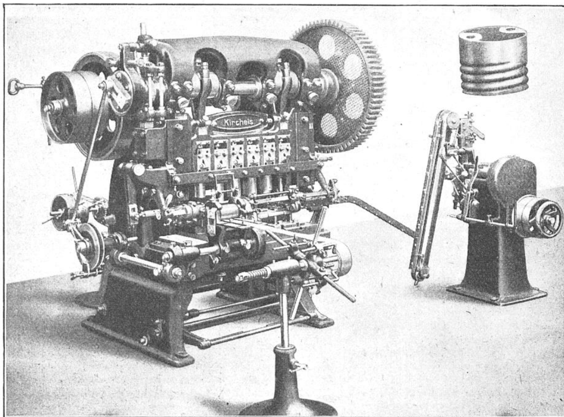
FIG. 5. — PRESSE A SIX POINÇONS ACCOUPLEE AVEC UNE MACHINE A FILETER, POUR LA FABRICATION DES DOUILLES DE LAMPES ÉLECTRIQUES A INCANDESCENCE
