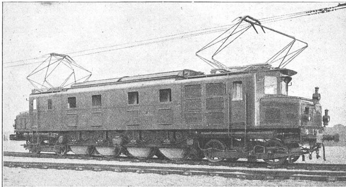
FIG. 6. — LOCOMOTIVE ÉLECTRIQUE A GRANDE VITESSE, DE 4.000 CH, DE LA COMPAGNIE DE PARIS-ORLÉANS. POIDS : 159 TONNES ; POIDS ADHÉRENT : 107 TONNES
