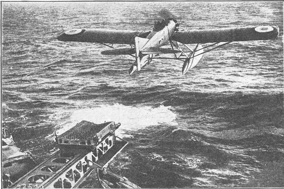
HYDRAVION « GOURDOU », A FLOTTEURS, PHOTOGRAPHIÉ AU MOMENT PRÉCIS OU IL QUITTE LE CHARIOT DE LA CATAPULTE DE LANCEMENT, A BORD D'UN BATIMENT DE GUERRE
