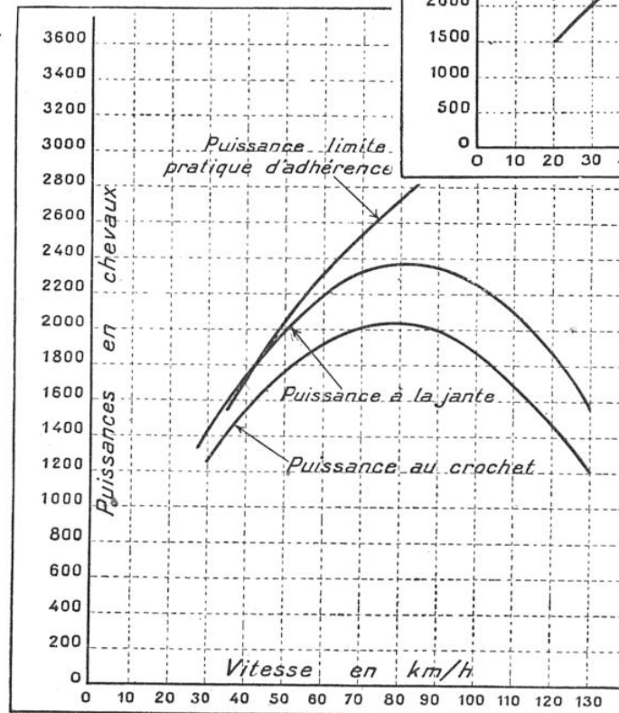
FIG. 3. — VARIATIONS DE LA PUISSANCE A LA JANTE D'UNE LOCOMOTIVE A VAPEUR, TYPE MOUNTAIN
