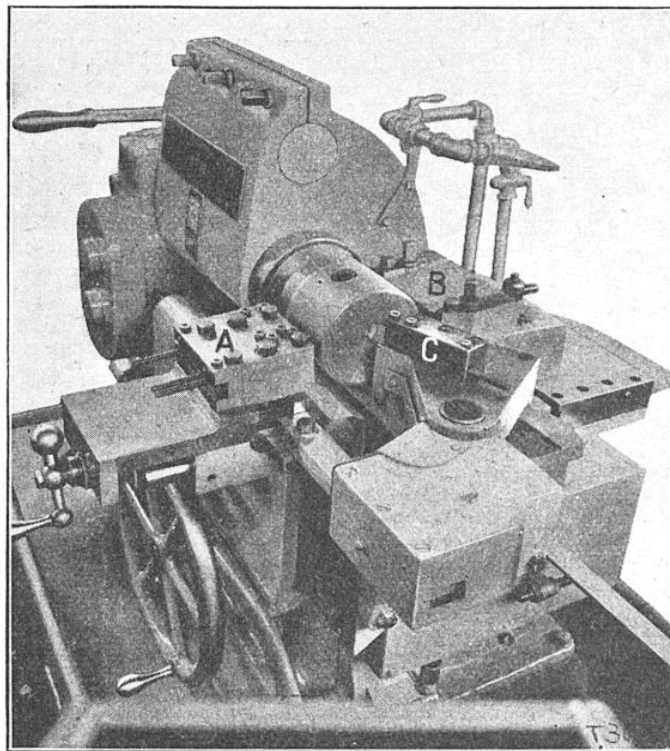
FIG. 3. — TOUR A UNE SEULE BROCHE EXÉCUTANT SIMULTANÉMENT PLUSIEURS OPÉRATIONS SUR UNE MÊME PIÈCE Les outils portés par les trois chariots A, B et C travaillent ensemble au cylindrage d'un piston en aluminium, à l'exécution des gorges de segments et au dressage du fond.
