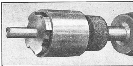
FIG. 10. — COMMENT S'EFFECTUE LE CONTRÔLE AUTOMATIQUE DE LA RECTIFICATION INTÉRIEURE
