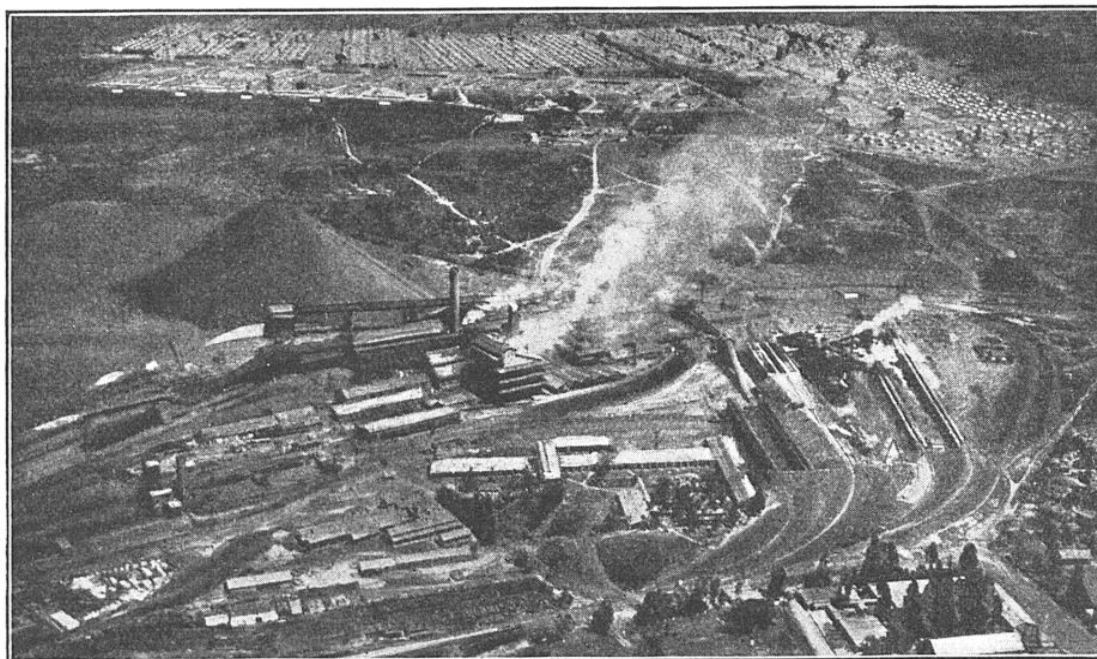
VUE AÉRIENNE DES USINES ÉQUIPÉES À LA MODERNE DE LUBUMBASHI (HAUT-KATANGA) Ces usines assurent le traitement du minerai de cuivre. On remarquera, dans le fond, les cités ouvrières pour les travailleurs indigènes employés dans cet important centre métallurgique.
