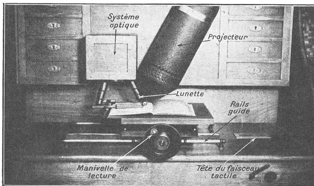
LA TABLE DU PHOTOÉLECTROGRAPHE
