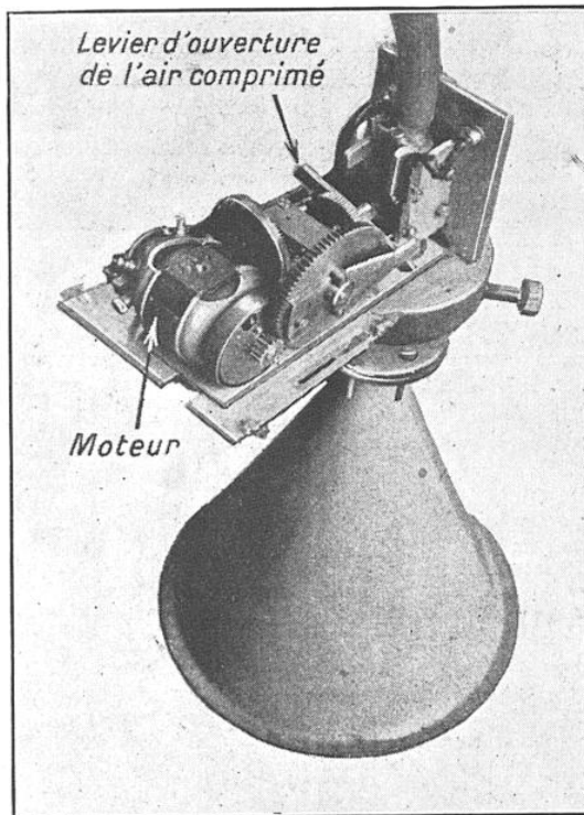
FIG. 4. — VIBRATEUR A AIR COMPRIMÉ POUR L'ÉMISSION DU SON
