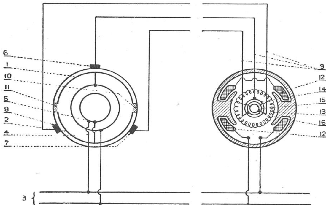
FIG. 5. — SCHÉMA DE PRINCIPE DE LA TRANSMISSION A DOUZE POSITIONS ST-CHAMOND-GRANAT A gauche, le transmetteur ; à droite, le récepteur, alimentés par la ligne 3, à courant continu ou alternatif. 1 et 2, bagues conductrices séparées par les isolants 10 et 11 ; 4 et 5, balais d'alimentation des bagues 1 et 2 ; 6, 7 et 8, balais alimentant le rotor 13 du récepteur par la ligne 9 et les bagues 14, 15, 16 ; 12, inducteur fixe du récepteur. Les balais 6, 7, 8 du transmetteur peuvent prendre, par rapport aux bagues 1 et 2 et aux isolants 10 et 11, douze positions différentes. La variation des potentiels sous ces balais fait varier le courant dans la ligne 9 et le champ résultant dans le rotor récepteur change de direction. Celui-ci prend donc une nouvelle position d'équilibre correspondant à la coïncidence de ce champ avec le champ inducteur fixe. Ainsi, à un ordre transmis correspond une seule indication du récepteur.
