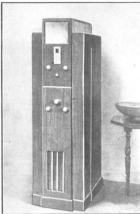
FIG. 9. — ENSEMBLE AMÉRICAIN COMPORTANT A LA FOIS UN RÉCEPTEUR DE TÉLÉVISION (EN HAUT) ET UN POSTE DE T. S. F. (EN BAS)
