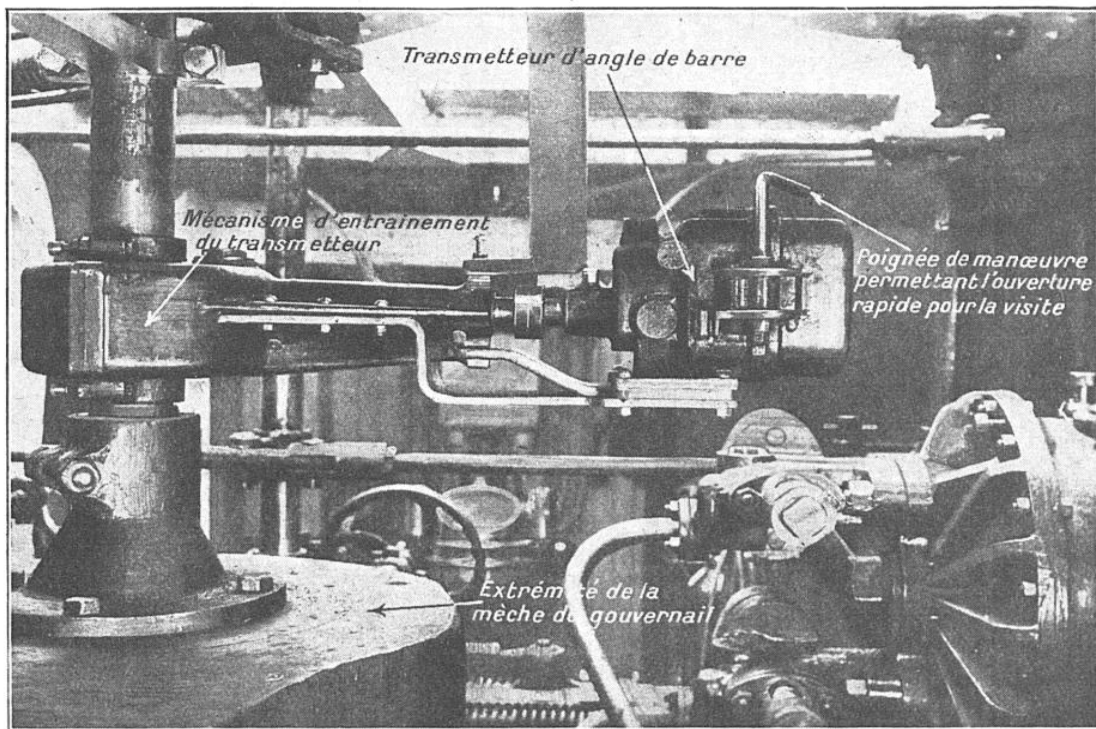
FIG. 8. — TRANSMETTEUR D'ANGLE DE BARRE AVEC SON MÉCANISME D'ENTRAÎNEMENT
