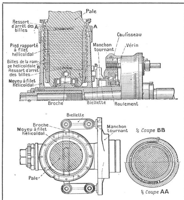
FIG. 3. — SCHÉMA DE L'HÉLICE A PAS VARIABLE « RATIER »
