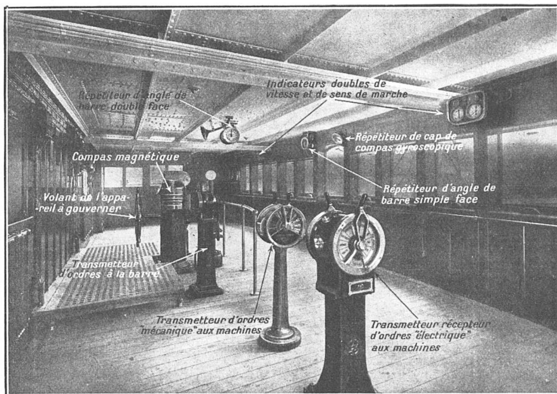
FIG. 1. — VUE D'ENSEMBLE DE LA PASSERELLE DU PAQUEBOT A CLASSE UNIQUE « CHAMPLAIN », RÉCEMMENT MIS EN SERVICE ENTRE LE HAVRE ET NEW YORK
