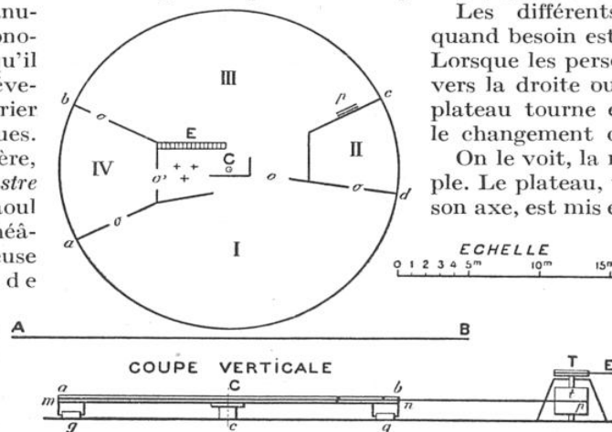
FIG. 2. — VUE EN PLAN ET COUPE VERTICALE SCHÉMATIQUES DE LA SCÈNE TOURNANTE DE L'OPÉRA DE PARIS. Le plateau a b c d est divisé en quatre parties I, II, III, IV, pour les décors de l' Illustre Fregona . AB figure le rideau. On voit sur la coupe le treuil T , sur lequel s'enroule le câble E qui fait tourner le plateau autour de l'axe C .
