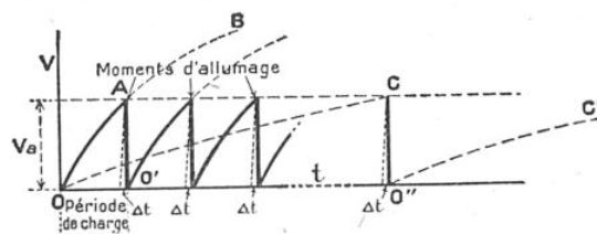
FIG. 24. — OSCILLATIONS EN « DENTS DE SCIE » OBTENUES AVEC LE SYSTÈME A RELAXATION. La courbe OAB est la courbe exponentielle de la charge du condensateur C. Au moment où la tension à ses bornes atteint la valeur d'allumage V_a , la lampe s'allume en déchargeant le condensateur dans un temps excessivement court \Delta t . \Delta t étant négligeable vis-à-vis du temps de charge, on peut considérer, dans la pratique, la décharge du condensateur comme instantanée.
