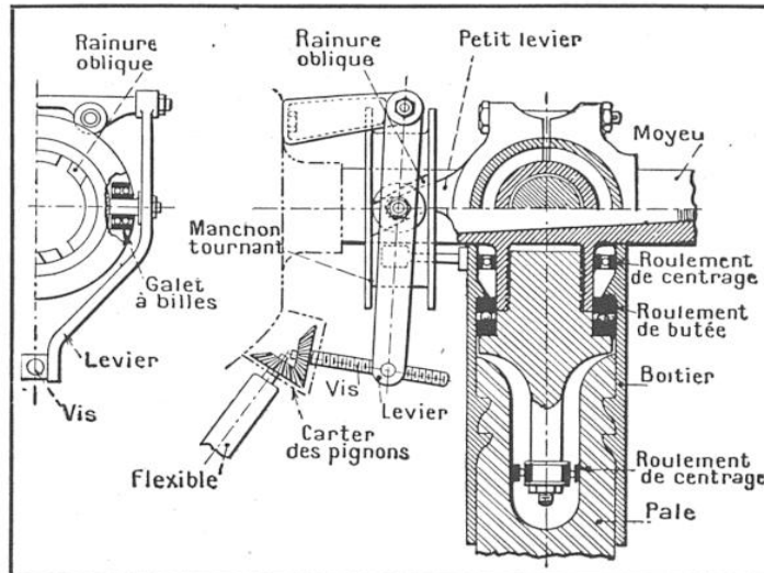
FIG. 8. — SCHÉMA DE FONCTIONNEMENT DE L'HÉLICE « CHAUVIÈRE »
