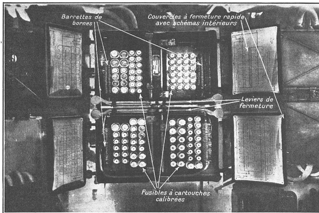
FIG. 10. — BOITE ÉTANCHE CONTENANT UN GRAND NOMBRE DE FUSIBLES ÉGALEMENT ÉTANCHES. Remarquer sur l'intérieur des portes de fermeture, le schéma des connexions établies par ces fusibles.
