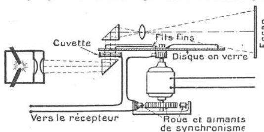
FIG. 26. — NOUVEAU TÉLÉVISEUR ORIGINAL DE L'AMÉRICAIN JENKINS
