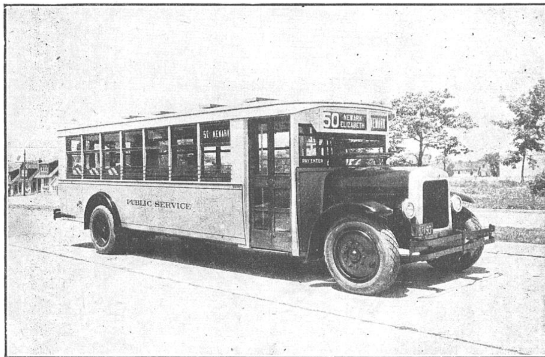
FIG. 4. — AUTOCAR AMÉRICAIN A TRANSMISSION « PÉTROLEO-ÉLECTRIQUE ». LE MOTEUR ENTRAÎNE UNE DYNAMO ALIMENTANT UN MOTEUR ÉLECTRIQUE A L'ARRIÈRE
