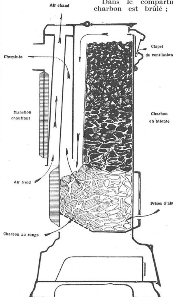
COUPE DU POÊLE « CINEY »
