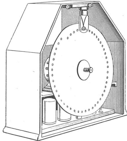
FIG. 19. — VUE ARRIÈRE D'UN TÉLÉVISEUR MODERNE AVEC ROUE A LENTILLES
