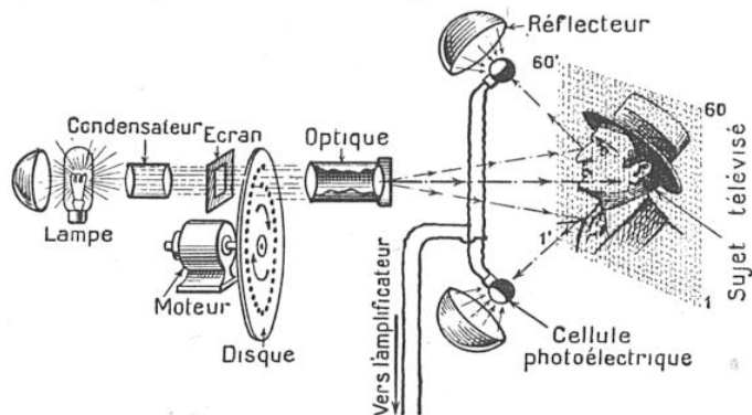
FIG. 3. — SYSTÈME D'EXPLORATION DE L'IMAGE DIT A « SPOT VOLANT »
