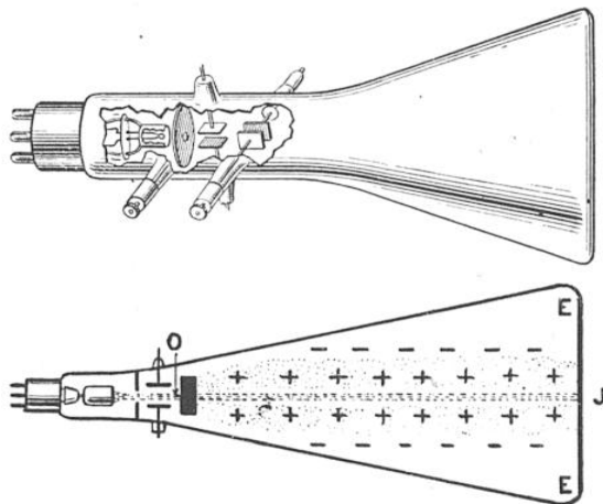
FIG. 20 ET 21. — LA TÉLÉVISION PAR RAYONS CATHODIQUES (TUBE DE BRAUN)
