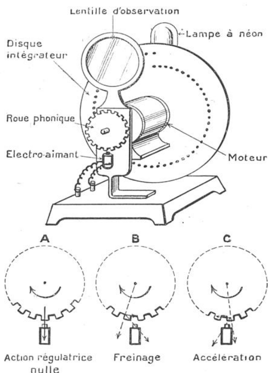
FIG. 7. — ENSEMBLE D'UN RÉCEPTEUR D'AMATEUR DONT LA VITESSE EST RÉGLÉE PAR UNE « ROUE PHONIQUE »
