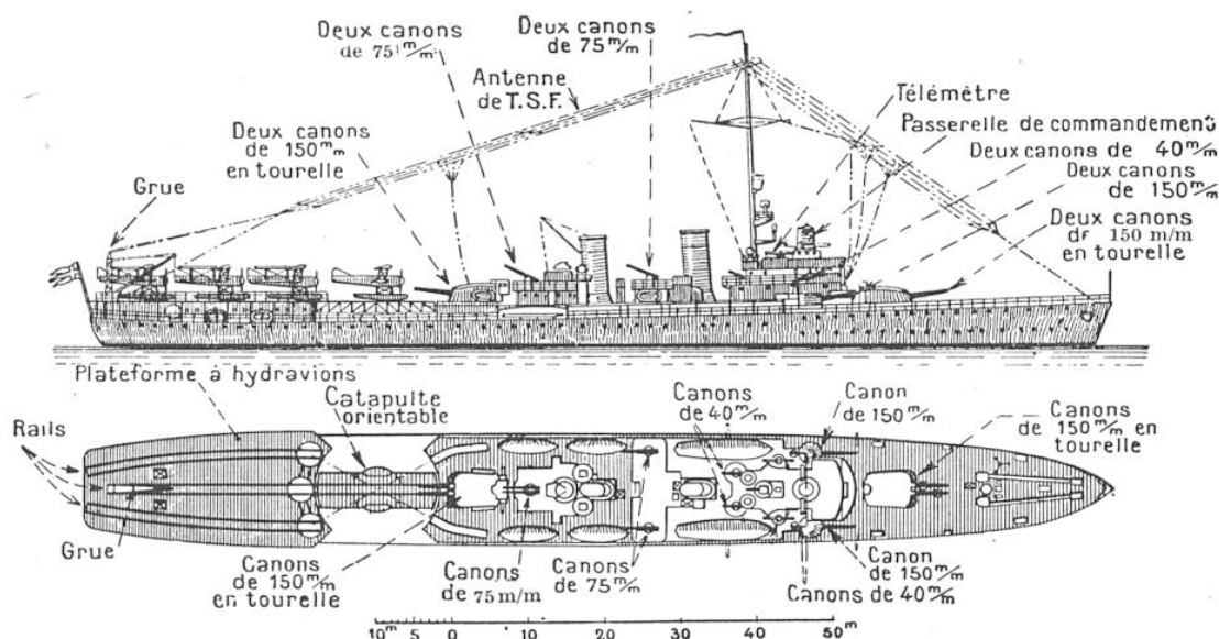
FIG. 3. — COMMENT LE « GOTLAND » EST ARMÉ ET ÉQUIPÉ
