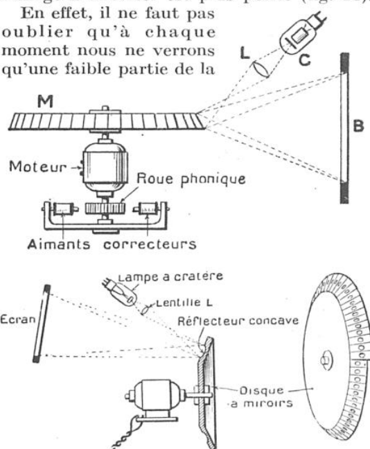
FIG. 16 ET 17. — TÉLÉVISEURS UTILISANT UNE ROUE A MIROIRS A LA PLACE DU DISQUE Les rayons issus de la lampe à cratère C sont concentrés par la lentille L et, après réflexion sur une des facettes de la roue à miroirs M, forment l'image du cratère sur l'écran B. Le nombre des miroirs est égal au nombre des bandes de l'analyse. On voit, en dessous, la forme de la roue à miroirs. Chaque miroir explore une bande de l'image, à la place des trous du disque de Nipkow.
