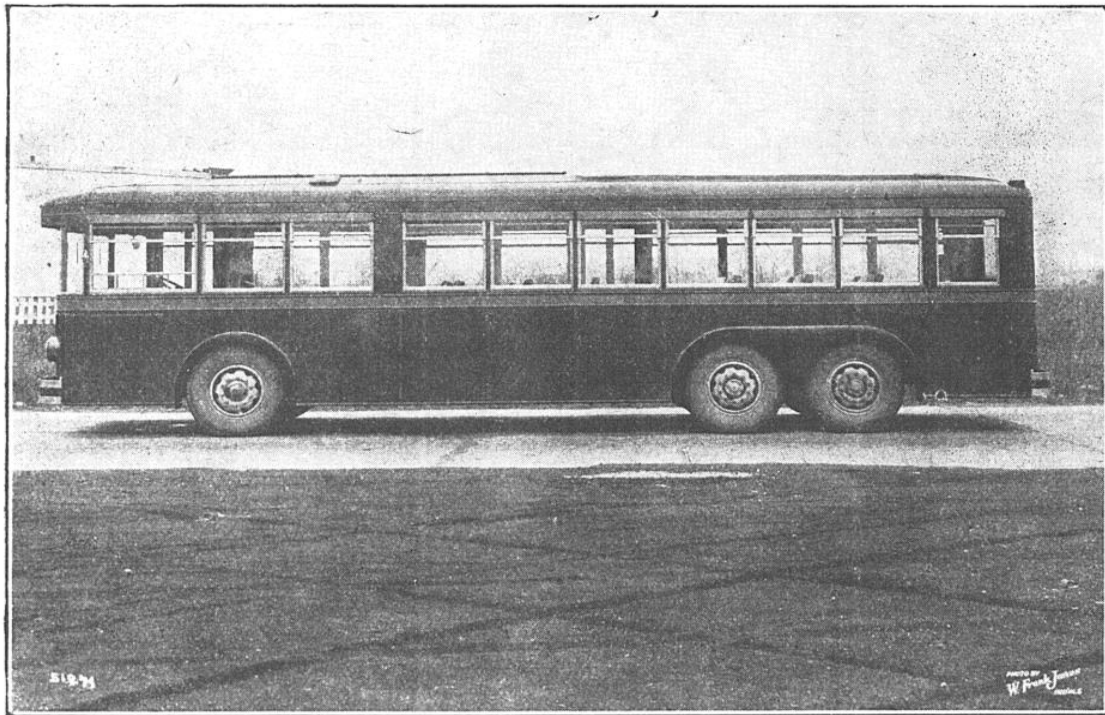
FIG. 3. — OMNIBUS A VAPEUR, DE 40 PLACES ET A SIX ROUES, EN USAGE AUX ÉTATS-UNIS
