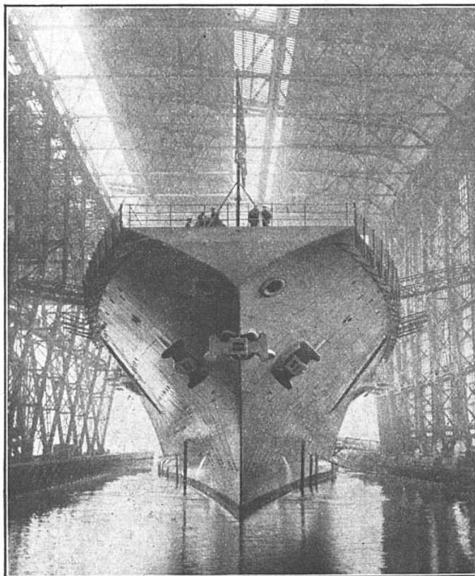
FIG. 8. — LE PORTE-AVIONS AMÉRICAIN « SARATOGA »
