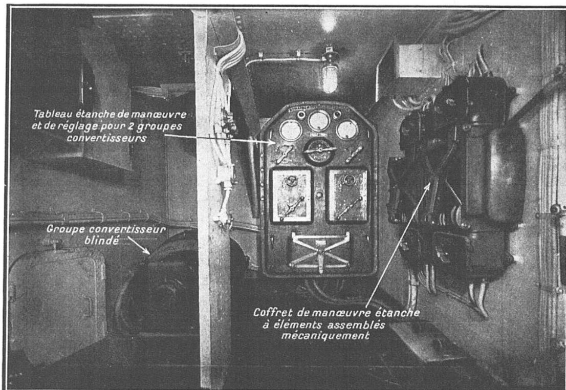
FIG. 9. — CE GROUPE CONVERTISSEUR BLINDÉ EST ÉQUIPÉ AVEC UN APPAREILLAGE ÉLECTRIQUE COMPLÈTEMENT ÉTANCHE, ABSOLUMENT À L'ABRI DES CORROSIONS DUES À L'HUMIDITÉ
