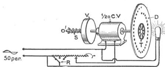
FIG. 5. — CONTRÔLE DE LA VITESSE DU DISQUE La vitesse du moteur est réglée par un rhéostat R. Le disque stroboscopique T, éclairé par un courant alternatif qui alimente le moteur, permet de contrôler si la vitesse est exacte. La résistance r assure la finition du réglage. Le volant V, monté sur un ressort S, régularise le mouvement.
