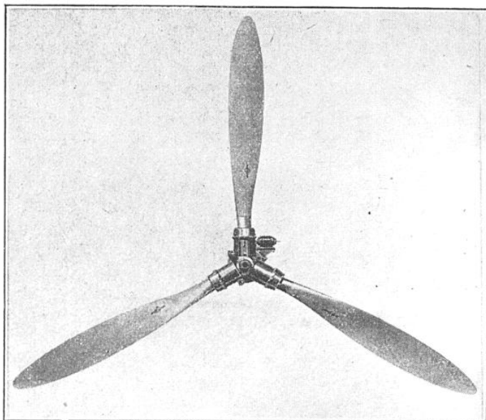
FIG. 6. — ENSEMBLE DE L'HÉLICE A PAS VARIABLE Cette hélice, dont le moyeu est représenté à plus grande échelle sur la page précédente, est destinée à l'avion stratosphérique Guerchais. (Voir La Science et la Vie, n° 178, page 273.)
