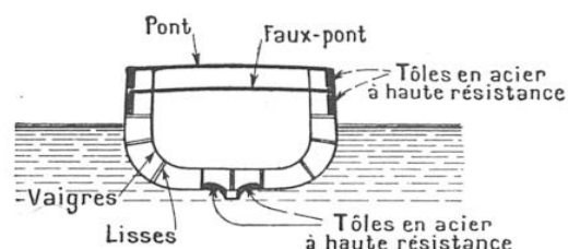
FIG. 2. — COMMENT EST CONSTITUÉE LA COQUE DU NOUVEAU NAVIRE LE « GOTLAND »
