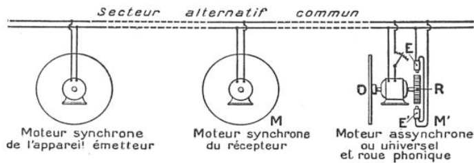
FIG. 10. — SYNCHRONISATION SEMI-AUTOMATIQUE DES RÉCEPTEURS DE TÉLÉVISION
