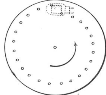
FIG. 12 ET 13. — LAMPE AU NÉON ET POSITION DE LA LAMPE DERRIÈRE LE DISQUE PERFORÉ
