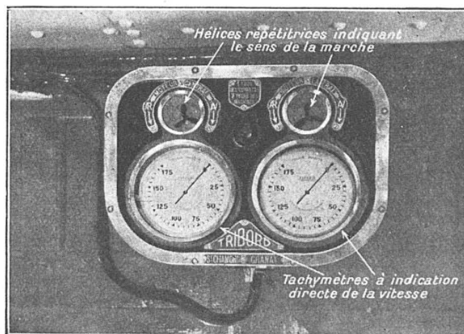
FIG. 2. — INDICATEUR DOUBLE DE VITESSE ET DE SENS DE MARCHE DES HÉLICES DU « CHAMPLAIN »
