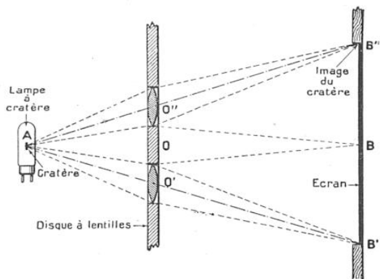
FIG. 18. — LE DISQUE A LENTILLES TEND A REMPLACER LE DISQUE A MIROIRS
