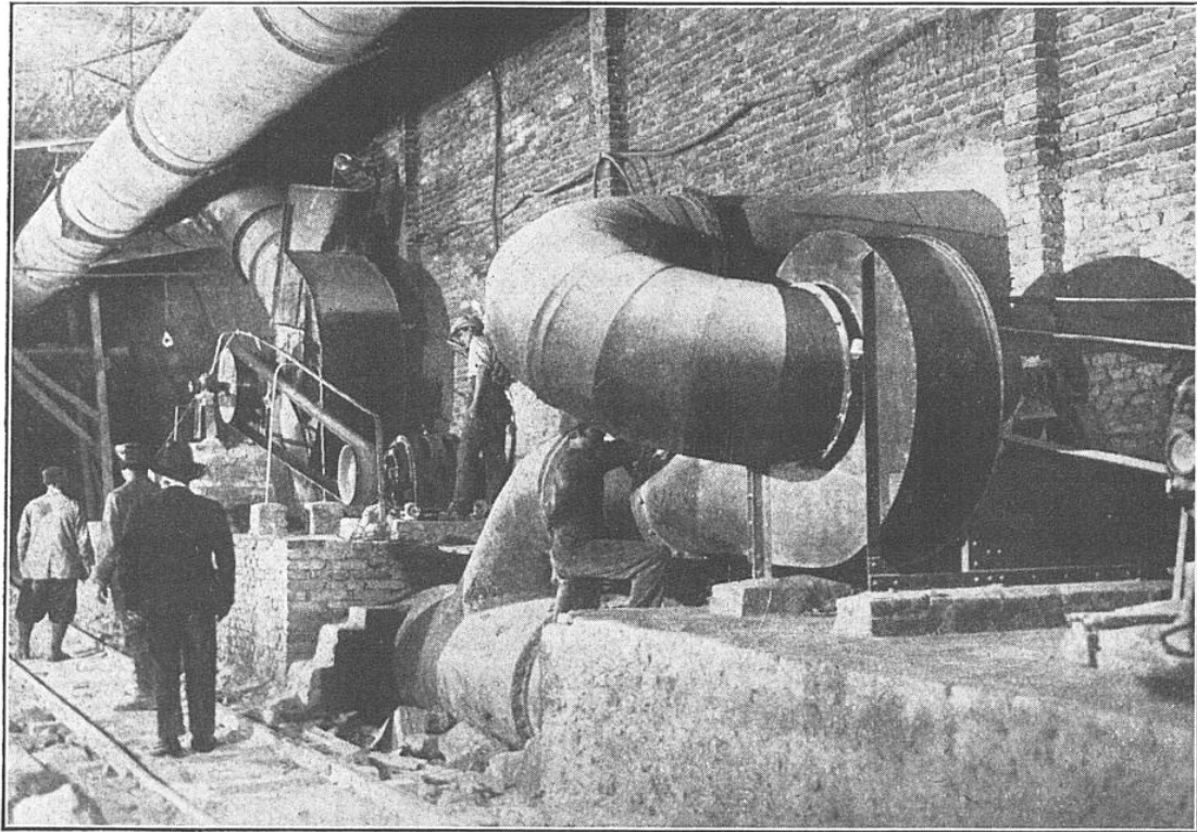
FIG. 3. - INSTALLATION DE VENTILATION POUR LE CREUSEMENT DU GRAND TUNNEL DE L'APENNIN L'air frais, amené par une conduite en maçonnerie, est repris par un ventilateur qui le refoule dans les tuyaux de tôle qui alimentent les parties les plus avancées du chantier.
