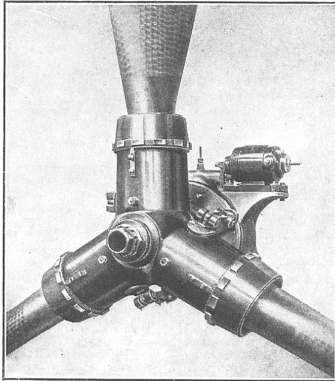
FIG. 5. — HÉLICE A TROIS PALES A PAS VARIABLE
