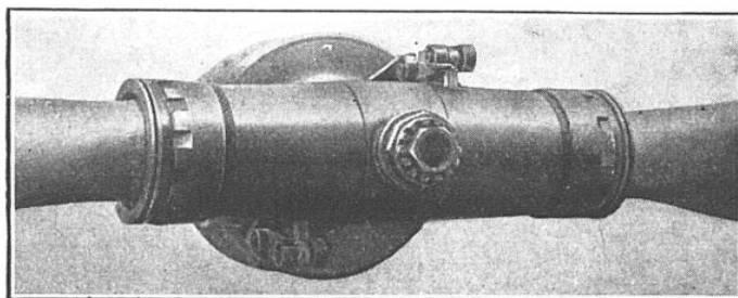
FIG. 4. — VUE DU MOYEU D'UNE HÉLICE A PAS VARIABLE « RATIER » A DEUX PALES
