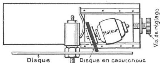
FIG. 6. — AUTRE MODE DE RÉGLAGE DE LA VITESSE DU DISQUE
