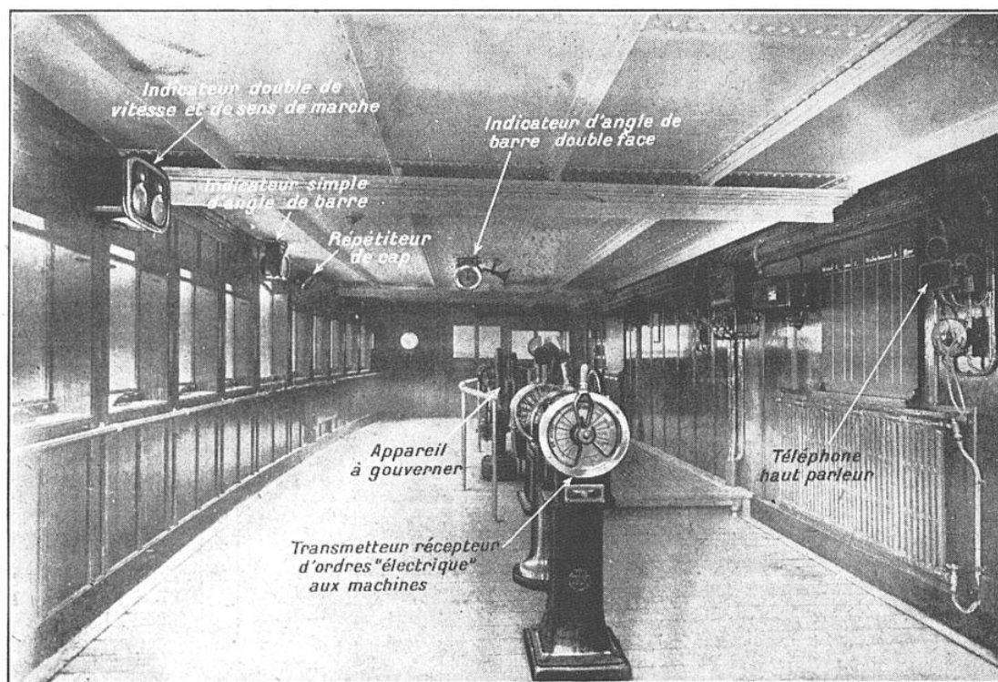
FIG. 4. — AUTRE VUE DE LA PASSERELLE DU « CHAMPLAIN », MONTRANT LES TÉLÉPHONES AVEC HAUT-PARLEURS POUR LA COMMUNICATION DES ORDRES AU MARIN SITUÉ SUR LA PASSERELLE. On retrouve ici les divers organes déjà signalés sur la figure 1.
