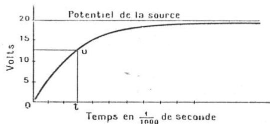
FIG. 8. — COURBE DE CHARGE D'UN CONDENSATEUR EN FONCTION DU TEMPS
