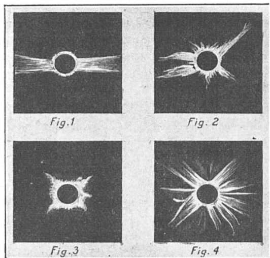
FIG. 1, 2, 3 ET 4. — DIFFÉRENTS ASPECTS QUE PREND LA COURONNE SOLAIRE AUX DIFFÉRENTES PÉRIODES D'ACTIVITÉ
