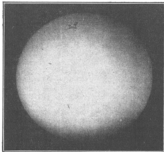
FIG. 5. — ASPECT DU DISQUE SOLAIRE On voit, à la partie supérieure, une grosse tache.
