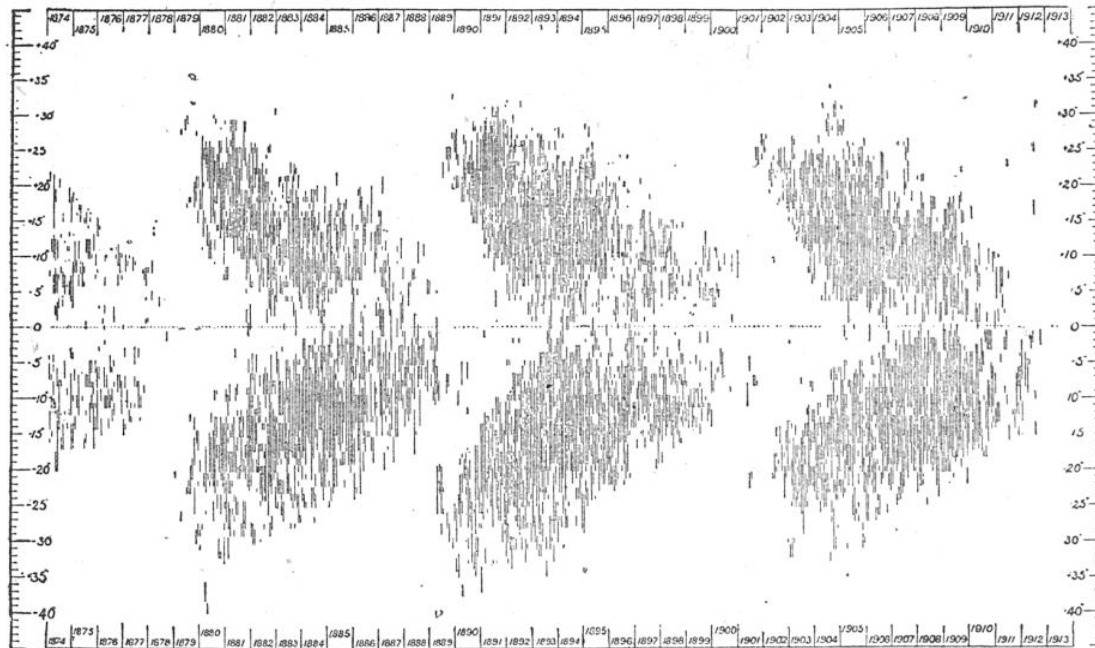
FIG. 8. — SCHÉMA MONTRANT LA VARIATION UNDÉCENNALE DE L'ACTIVITÉ SOLAIRE
