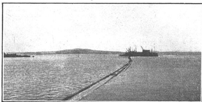
FIG. 4. — COMMENT ON PROCÈDE A LA POSE DE LA PIPE-LINE Les conduites sont hermétiquement bouchées. Pour les immerger, on les remplit d'eau.
