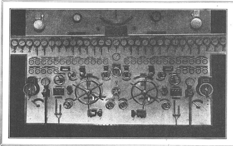
PAQUEBOT CHAMPLAIN, DE LA COMPAGNIE GÉNÉRALE TRANSATLANTIQUE Vue du tableau de manœuvre de la salle des machines montrant les appareils récepteurs transmetteurs d'ordres.
