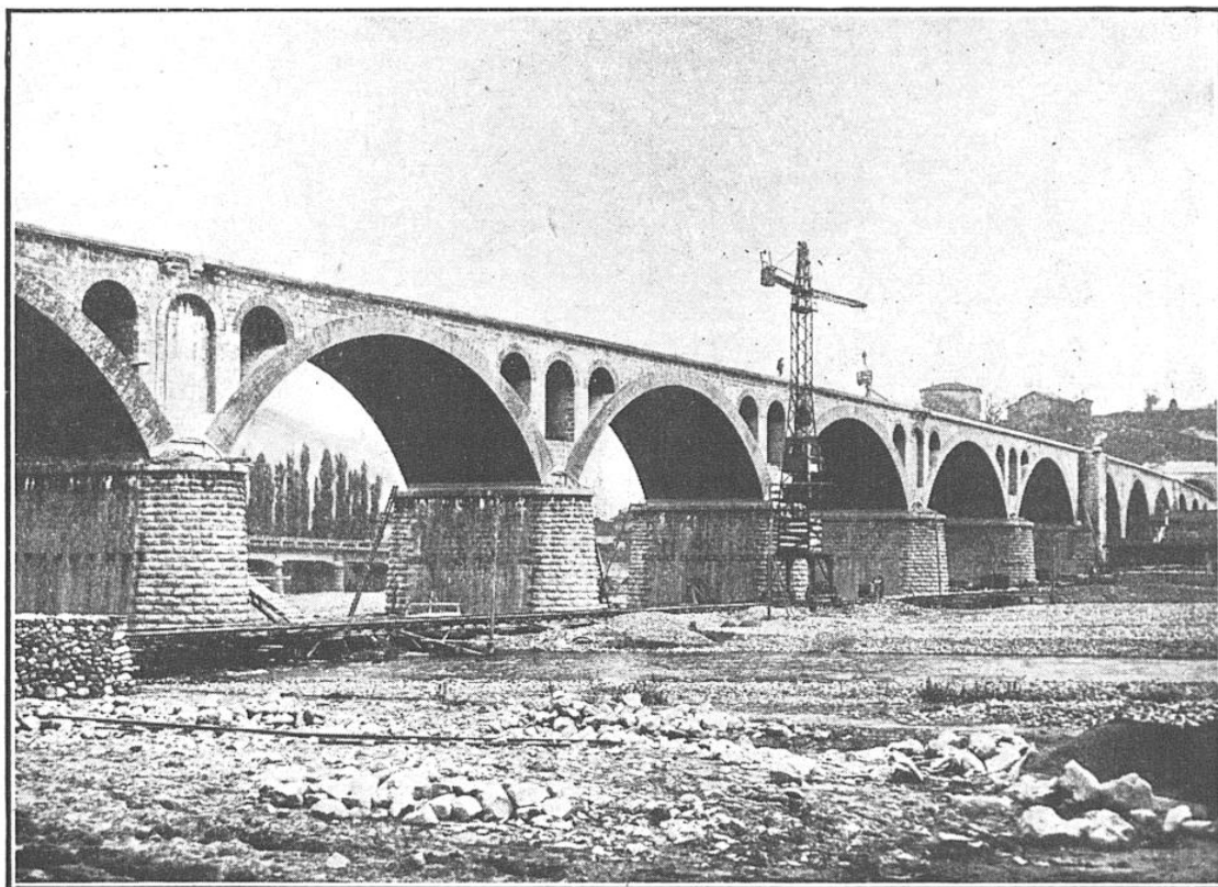
FIG. 2. — VUE D'ENSEMBLE DU PONT-VIADUC ÉTABLI POUR LA TRAVERSÉE DU TORRENT SETTA, PRÈS DE VADO, A 15 KILOMÈTRES AU SUD DE BOLOGNE
