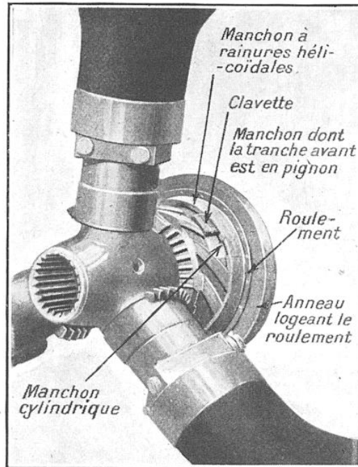
FIG. 1. — MOYEU D'UNE HÉLICE A TROIS PALES A PAS VARIABLE « FUSCALDO »
