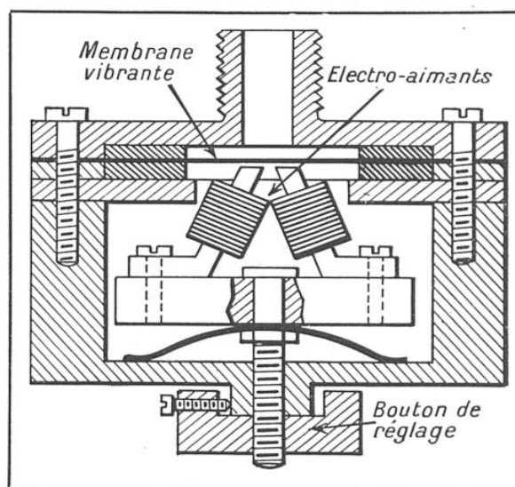
FIG. 5. — MICROPHONE RÉCEPTEUR A MEMBRANE
