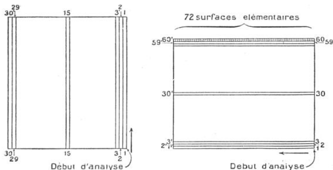
FIG. 1. — L'EXPLORATION DE L'IMAGE EST L'OPÉRATION FONDAMENTALE DE LA TÉLÉVISION
