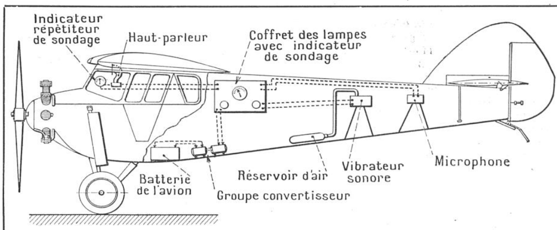
FIG. 9. — SCHÉMA D'UN AVION ÉQUIPÉ AVEC UN APPAREIL DE SONDAGE ACOUSTIQUE
