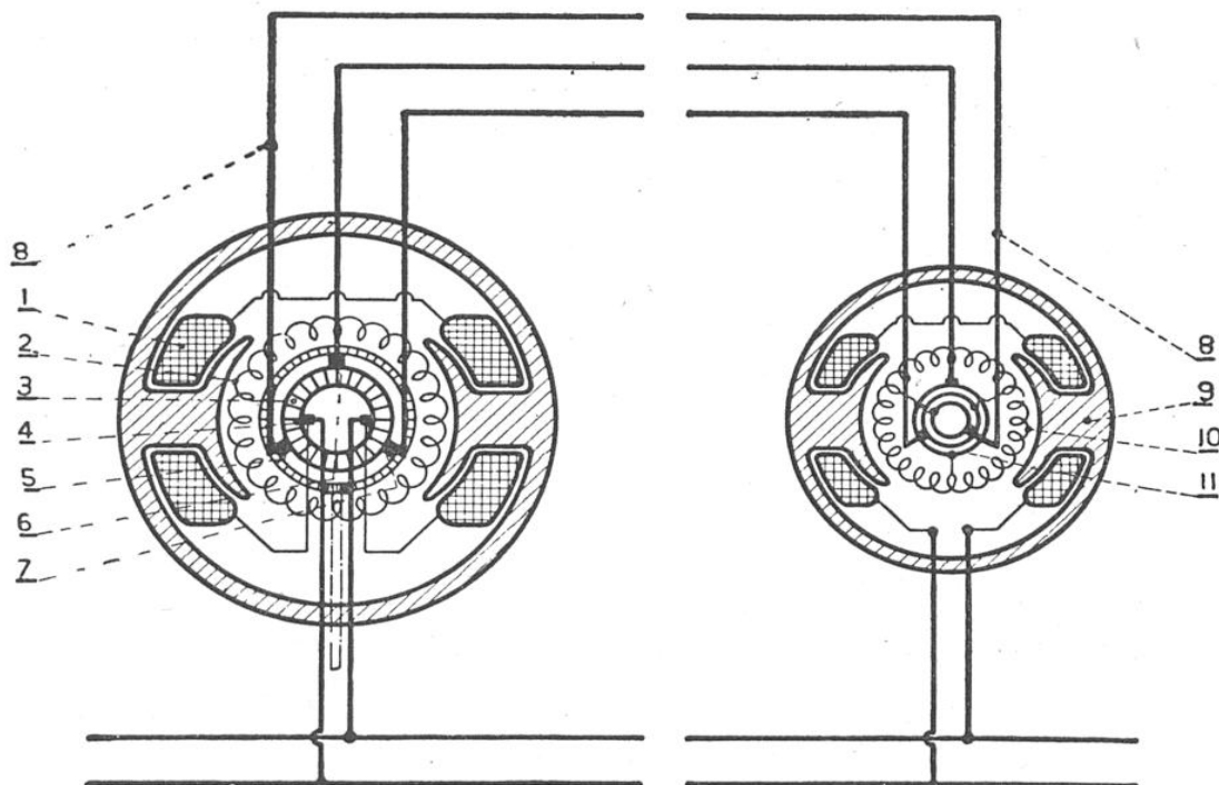
FIG. 6. — SCHÉMA PERMETTANT DE COMPRENDRE LE PRINCIPE DE LA TRANSMISSION ÉLECTRIQUE À INDICATIONS CONTINUES SAINT-CHAMOND-GRANAT
