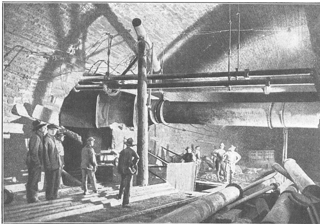
FIG. 4. — L'ABOUTISSEMENT AU NIVEAU DE LA VOIE FERRÉE, A 270 MÈTRES DE PROFONDEUR, D'UN DES DEUX Puits INCLINÉS, CREUSÉS POUR ATTAQUER LE TUNNEL PAR LE CENTRE On voit le gros tuyau de ventilation et les tuyaux plus petits pour l'évacuation de l'eau.
