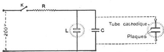
FIG. 23. — SCHÉMA D'UN DISPOSITIF, DIT A « RELAXATION », QUI ASSURE LE BALAYAGE DE L'ÉCRAN PAR LA TACHE CATHODIQUE. Fermons l'interrupteur K. Le condensateur C se charge à travers une forte résistance R. Cette charge sera d'autant plus longue que la résistance R sera plus forte et que la capacité du condensateur C sera plus grande. Plaçons une lampe à incandescence L en parallèle avec le condensateur C. On sait que les lampes à incandescence s'allument brusquement dès que le voltage à leurs bornes atteint une certaine valeur minimum dite « tension d'allumage ». Donc, dès que la tension aux bornes du condensateur C atteindra la « tension d'allumage », la lampe L s'allumera. Consommant un courant considérable, elle épuisera instantanément la réserve d'électricité accumulée dans le condensateur C et s'éteindra, ne pouvant pas recevoir assez de courant pour son fonctionnement à travers la résistance R. Dès que la lampe sera éteinte, la charge du condensateur C commencera automatiquement jusqu'au nouvel allumage de la lampe, et ainsi de suite. En faisant varier les valeurs de la résistance R et de la capacité C, nous pouvons faire varier dans de très larges limites la fréquence du phénomène dont la courbe 24 montre l'aspect.
