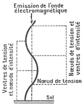
FIG. 1. — LES ONDES ÉLECTROMAGNÉTIQUES NE PEUVENT PAS SERVIR AU SONDAGE AÉRIEN
