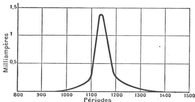
FIG. 6. — LE MICROPHONE NE FONCTIONNE QU'ENTRE DE FAIBLES LIMITES DE FRÉQUENCE
