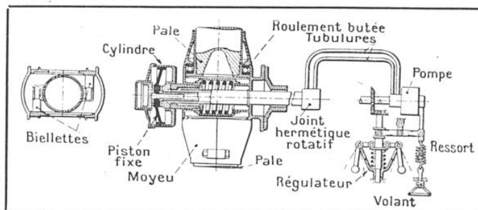
FIG. 7. — SCHÉMA DE FONCTIONNEMENT DE L'HÉLICE A PAS VARIABLE AUTOMATIQUEMENT « HELE-SCHAW »
