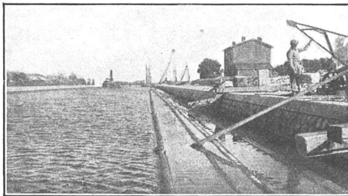
FIG. 3. - COMMENT SE FAIT LA MISE A L'EAU DE LA PIPE-LINE La photographie montre la mise à l'eau des quatre tronçons, d'une longueur totale de 535 mètres, pour la partie sous-marine de la conduite.
