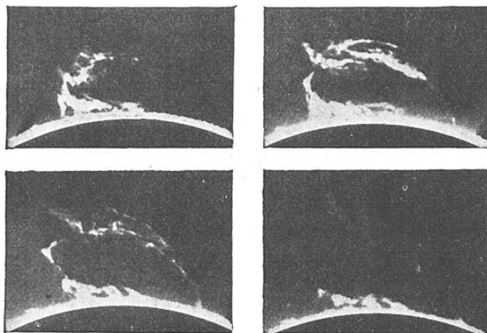
FIG. 11. — ÉVOLUTION RAPIDE D'UNE PROTUBÉRENCE SOLAIRE ENREGISTRÉE AU SPECTROHÉLIOGRAPHIE
