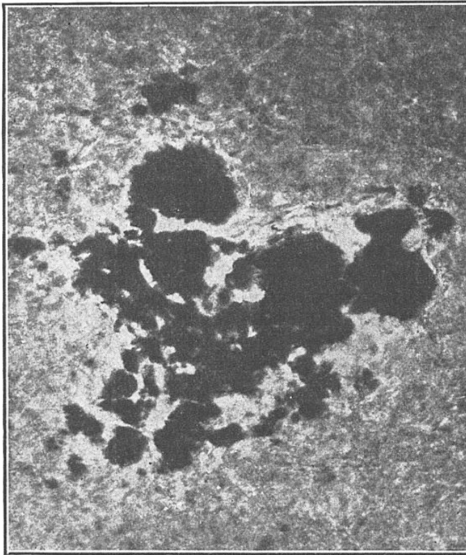
FIG. 7. — UN BEL « ARCHIPEL » DE TACHES SOLAIRES
