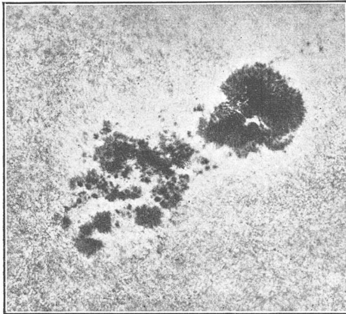
FIG. 6. — GROUPE DE TACHES SOLAIRES EN « ARCHIPEL » La plus grande de ces taches (en haut et à droite de la photo) a un diamètre très supérieur à celui de la Terre.
