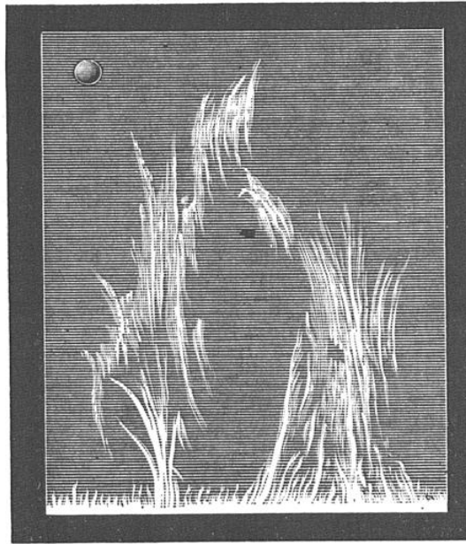
FIG. 10. — PROTUBÉRANCES SOLAIRES
