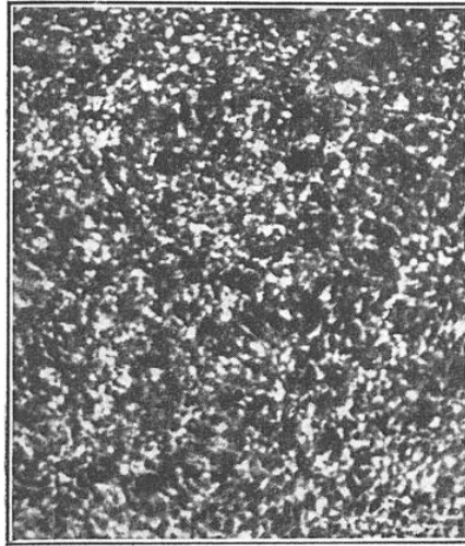
FIG. 9. — ASPECT DE LA SURFACE DU SOLEIL EN « GRAINS DE RIZ »
