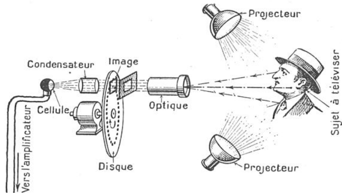
FIG. 2. — SYSTÈME « DIRECT » DE TÉLÉVISION
