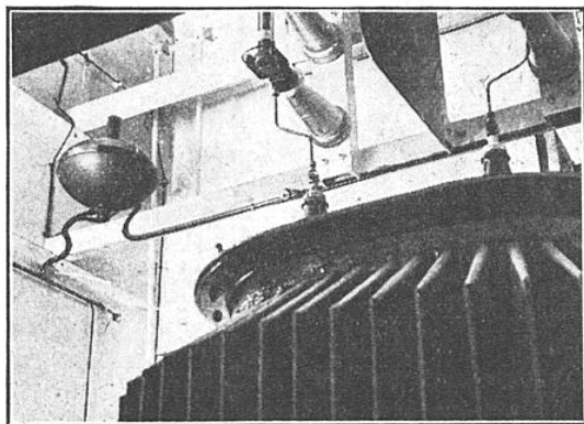
FIG. 2. -- PARTIE SUPÉRIEURE D'UN TRANSFORMATEUR DE LA CABINE HAUTE TENSION A gauche, l'extincteur « Assuro ».
