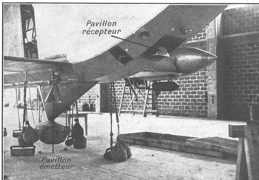
DISPOSITION DES APPAREILS DE SONDAGE SOUS LA NACELLE DU DIRIGEABLE
