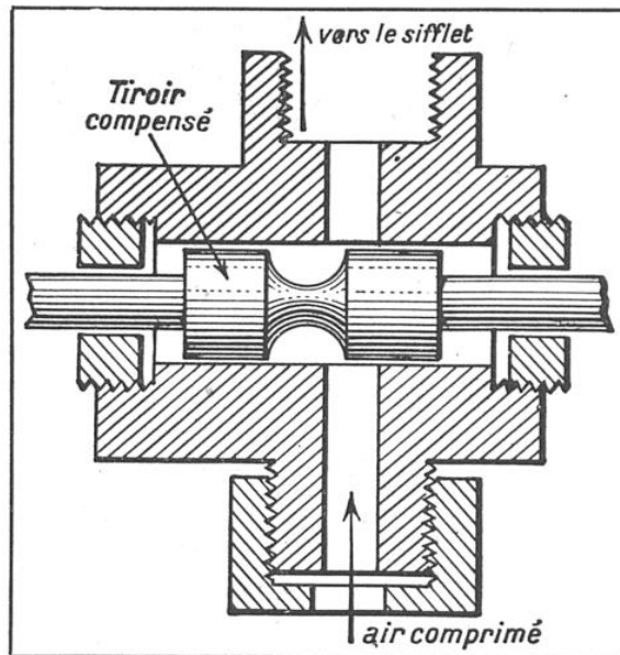
FIG. 3. — COMMENT ON DONNE UN COUP DE SIFFLET DURANT UN TEMPS TRÈS COURT
