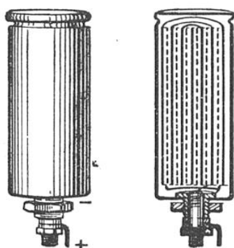
FIG. 5. — VUE ET COUPE D'UN CONDENSATEUR ÉLECTROLYTIQUE MODERNE
