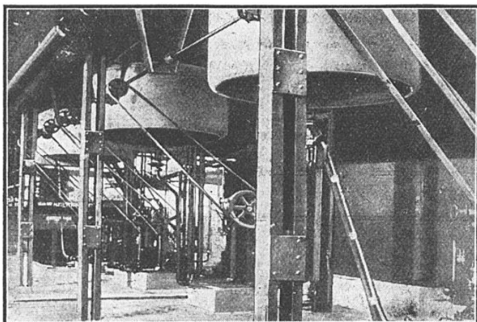
FIG. 1. — BROYEURS DE MINÉRAIS RADIFÈRES A L'USINE D'OOLEN PRÈS D'ANVERS (BELGIQUE)
