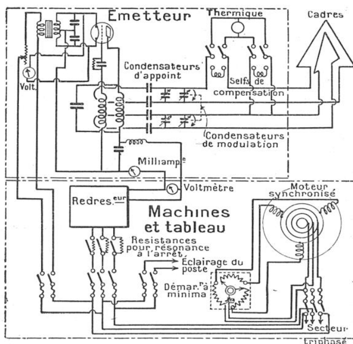
FIG. 4. — SCHÉMA DE PRINCIPE DE L'ENSEMBLE DU MONTAGE DU NOUVEAU RADIOPHARE INSTALLÉ AU BOURGET
