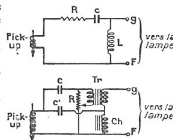
FIG. 23. — SCHÉMAS DE LIAISON D'UN PICK-UP AU POSTE RÉCEPTEUR
