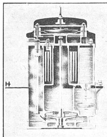
FIG. 7. DISJONCTION AUTOMATIQUE
