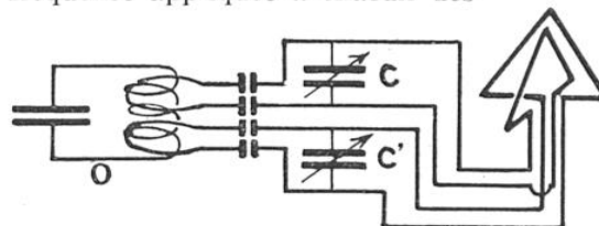
FIG. 3. — PRINCIPE D'ÉMISSION DU NOUVEAU RADIOPHARE DU BOURGET, PRÈS PARIS
