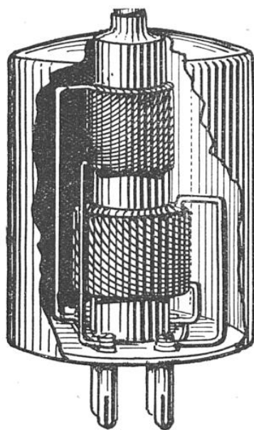
FIG. 14. — TYPE DE FILTRE D'UN RÉCEPTEUR MODERNE
