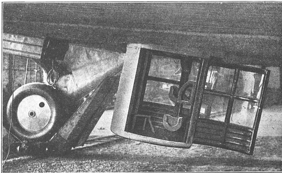
FIG. 5. — TOURELLE INFÉRIEURE DE L'AVION « S. A. B. 70 »
