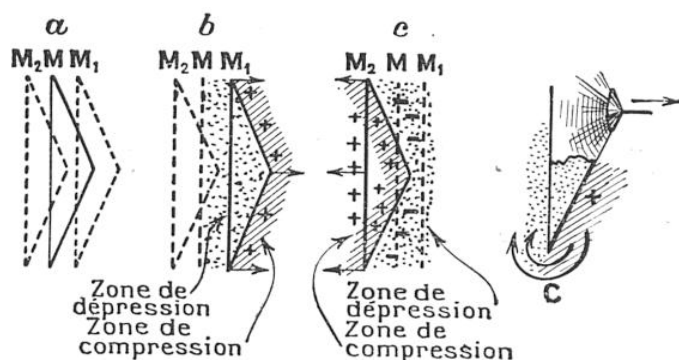
FIG. 21. — COMMENT SE PRODUIT LE PHÉNOMÈNE DU « COURT-CIRCUIT ACOUSTIQUE » DANS LES HAUT-PARLEURS À DIFFUSEURS
