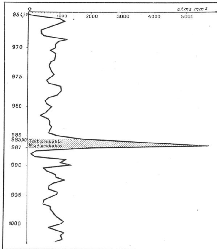
FIG. 13. -- LE SONDAGE ÉLECTRIQUE PERMET DE DÉCELER ET DE SITUER LES COUCHES DE HOUILLE
