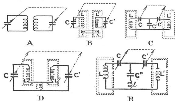
FIG. 15. — QUELQUES TYPES DE « FILTRES DE BANDES » UTILISÉS DANS LES POSTES DE T. S. F.
