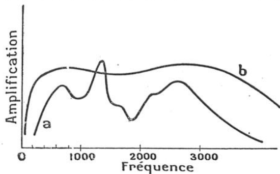
FIG. 18. — COURBES D'AMPLIFICATION DE TRANSFORMATEURS BASSE FRÉQUENCE
