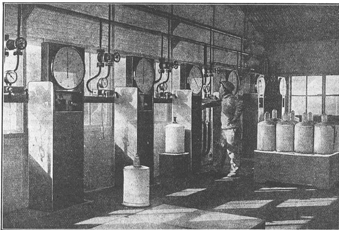
FIG. 8. — SALLE DES BALANCES ET DU REMPLISSAGE A L'USINE DE PETIT-COURONNE
