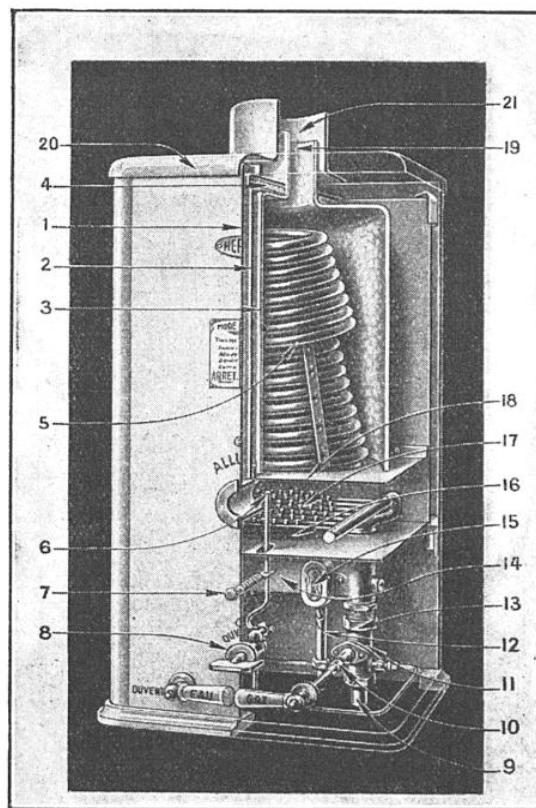
VUE EN COUPE DE « L'HERMINE »
