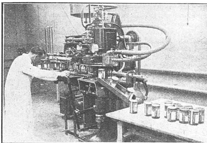
FIG. 9. — SERTISSAGE AUTOMATIQUE DES BOÎTES SOUS VIDE
