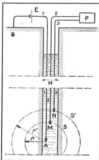
FIG. 4. COMMENT ON MESURE LES RÉSISTIVITÉS DANS UN SON- DAGE
