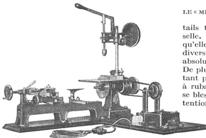
LE « MESOUTIL » AVEC TOUS SES ACCESSOIRES
