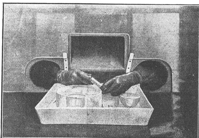
FIG. 8. — LA MANIPULATION DU RADIUM EN DEÇA DE L'ÉCRAN PROTECTEUR EN VERRE SPÉCIAL (FIG. 7) Les mains de l'opérateur exposées aux radiations sont gantées de caoutchouc épais mélangé avec de la limaille de plomb.
