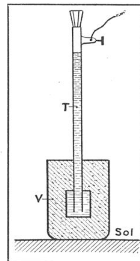
FIG. 3. — COMMENT EST CONSTITUÉE UNE ÉLECTRODE IMPOLARISABLE
