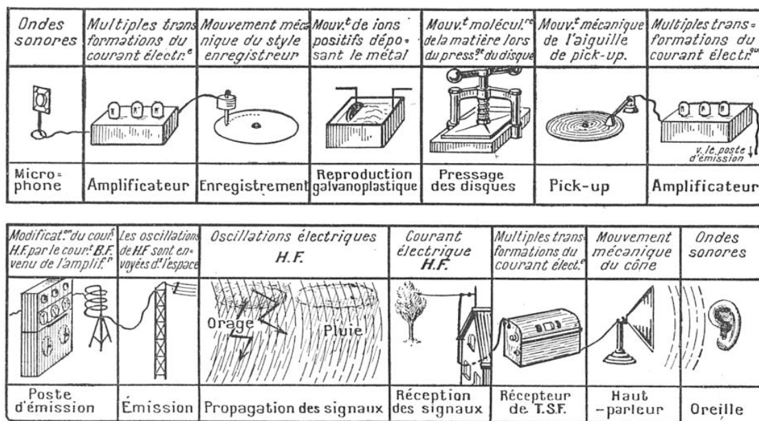
FIG. 1. — DE L'ÉMISSION À LA RÉCEPTION, LES CAUSES DE DÉFORMATION SONT NOMBREUSES. ELLES SONT SCHÉMATISÉES ICI POUR LE CAS DE LA TRANSMISSION DE LA MUSIQUE ENREGISTRÉE
