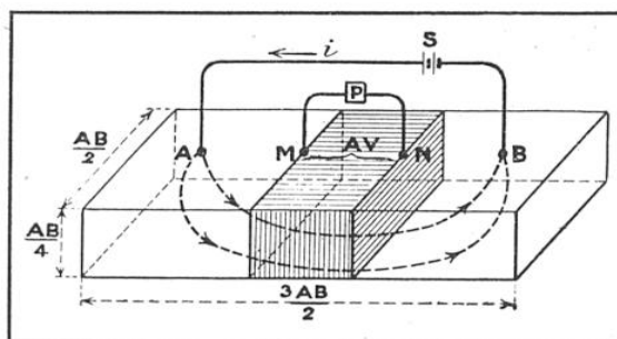
FIG. 1. — ÉTABLISSEMENT D'UNE CARTE DE RÉSISTIVITÉ ÉLECTRIQUE D'UN TERRAIN
