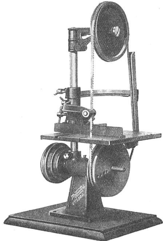
LE « MESOUTIL » UTILISÉ COMME SCIE A RUBAN
