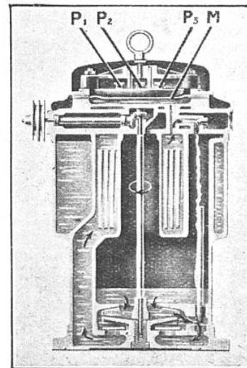
FIG. 4. RHÉOSTAT EN FIN DE DÉMARRAGE APRÈS EXÉCUTION DE LA MISE EN COURT-CIRCUIT
