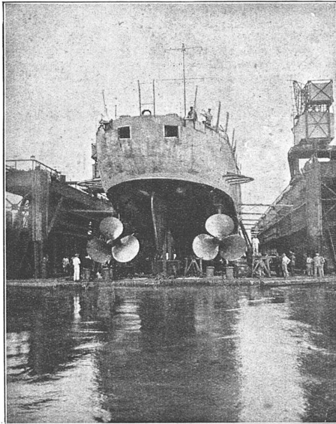
FIG. 5. - LE « CASSARD », EN CALE SÈCHE, VU DE L'ARRIÈRE On a adopté, pour les contre-torpilleurs de ce type, le modèle d'arrière dit « de croiseur ».
