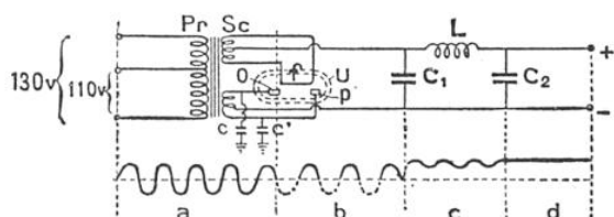
FIG. 2. — SCHÉMA D'UN DISPOSITIF D'ALIMENTATION D'UN RÉCEPTEUR PAR LE SECTEUR. Ce dispositif comprend un transformateur Pr Sc, une valve U, des condensateurs C_1 C_2 , une self L. Au-dessous, en a, b, c, d, formes du courant après son passage dans les différents organes.
