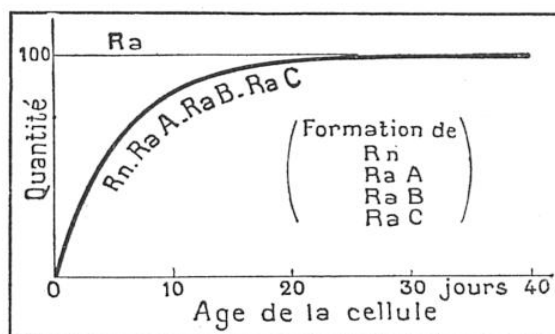
FIG. 12. — COURBE MONTRANT COMMENT UNE CELLULE DE RADIUM NE PARVIENT QUE PROGRESSIVEMENT (AU BOUT DE 25 JOURS) A SON « ÉTAT D'ÉQUILIBRE »
