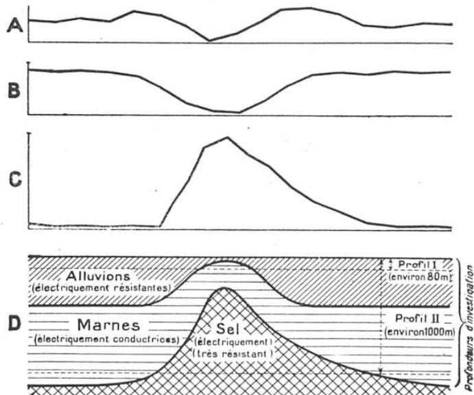
FIG. 10. — COMPARAISON DES MÉTHODES DE PROSPECTION ÉLECTRIQUE ET DES MÉTHODES GRAVIMÉTRIQUES
