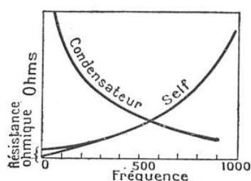
FIG. 4. — UNE SELF PRÉSENTE UNE RÉSISTANCE CROISSANTE AVEC LA FRÉQUENCE, TANDIS QU'UN CONDENSATEUR PRÉSENTE UNE RÉSISTANCE DÉCROISSANTE AVEC LA FRÉQUENCE DU COURANT
