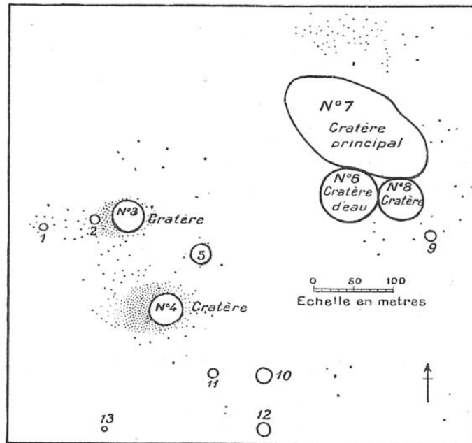
FIG. 5. — CARTE MONTRANT LA DISTRIBUTION DES CRATÈRES DE HENBURG (AUSTRALIE)
