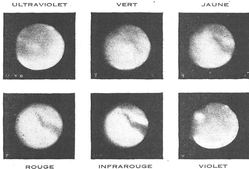
FIG. 10. — LA PHOTOGRAPHIE EN LUMIÈRE MONOCHROMATIQUE, AVEC DES PLAQUES SPÉCIALES, EST D'UN GRAND INTÉRÊT EN ASTRONOMIE, EN PARTICULIER POUR L'ÉTUDE DES PLANÈTES
