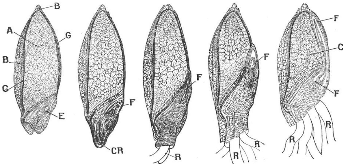
FIG. 1. — TRANSFORMATION DU GRAIN D'ORGE PENDANT LA GERMINATION
