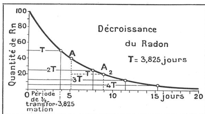
FIG. 11. — COURBE DE DÉSINTÉGRATION DU RADON
