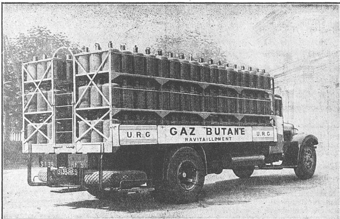
FIG. 4. — CAMION DE 8 TONNES SPÉCIALEMENT ÉQUIPÉ POUR LE TRANSPORT DU « BUTANE »
