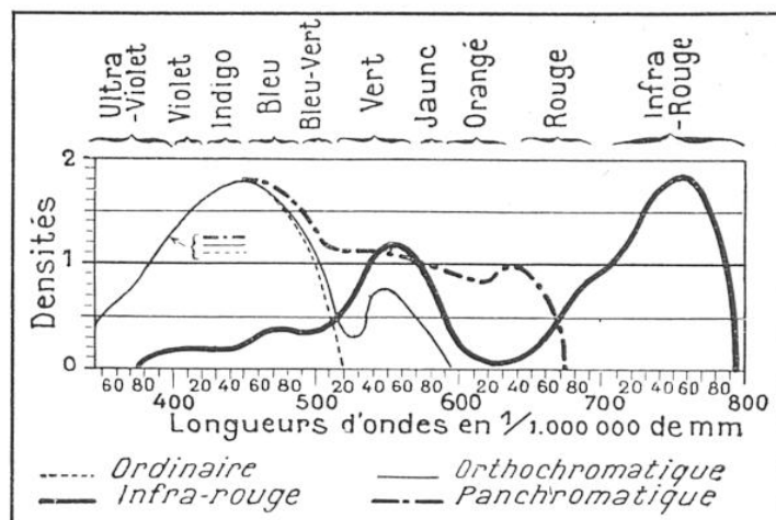
FIG. 3. — DIAGRAMME COMPARATIF MONTRANT LES SENSIBILITÉS DES DIVERSES SORTES DE PLAQUES (ORDINAIRES, ORTHOCHROMATIQUES, PANCHROMATIQUES ET SPÉCIALES POUR RAYONS INFRAROUGES) AUX VIBRATIONS LUMINEUSES DE DIFFÉRENTES LONGUEURS D'ONDES
