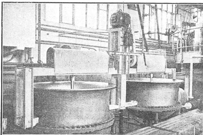
FIG. 7. — MALAXEURS DE CUIVRE OU S'OPÈRE LE MÉLANGE EXTRAIT DE MALT, LAIT, CACAO
