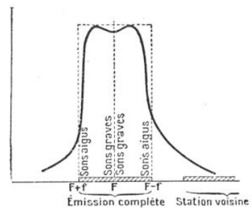
FIG. 13. — LA COURBE DE RÉSONANCE D'UN POSTE MODERNE SE RAPPROCHE DE LA COURBE PARFAITE DE LA FIGURE 12
