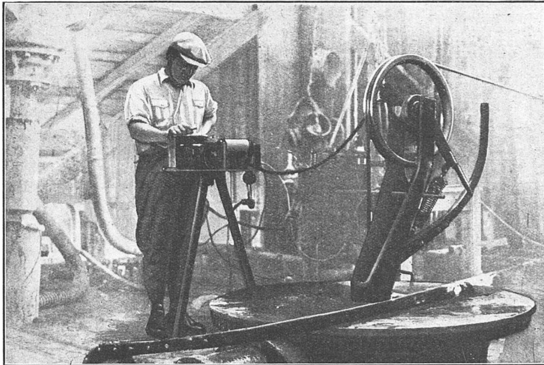
FIG. 6. — COMMENT ON PROCÈDE A UN « CAROTTAGE » ÉLECTRIQUE
