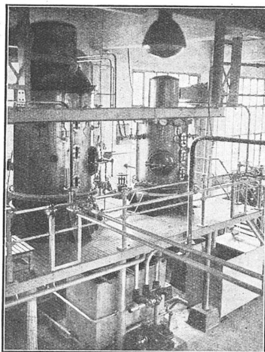
FIG. 6. — ÉVAPORATEURS UTILISÉS POUR PRÉPARER L'EXTRAIT DE MALT (A GAUCHE) ET POUR DÉSHYDRATER LE MÉLANGE EXTRAIT DE MALT, LAIT, JAUNE D'ŒUFS ET CACAO (A DROITE) VENANT DES MALAXEURS (FIG. 7)
