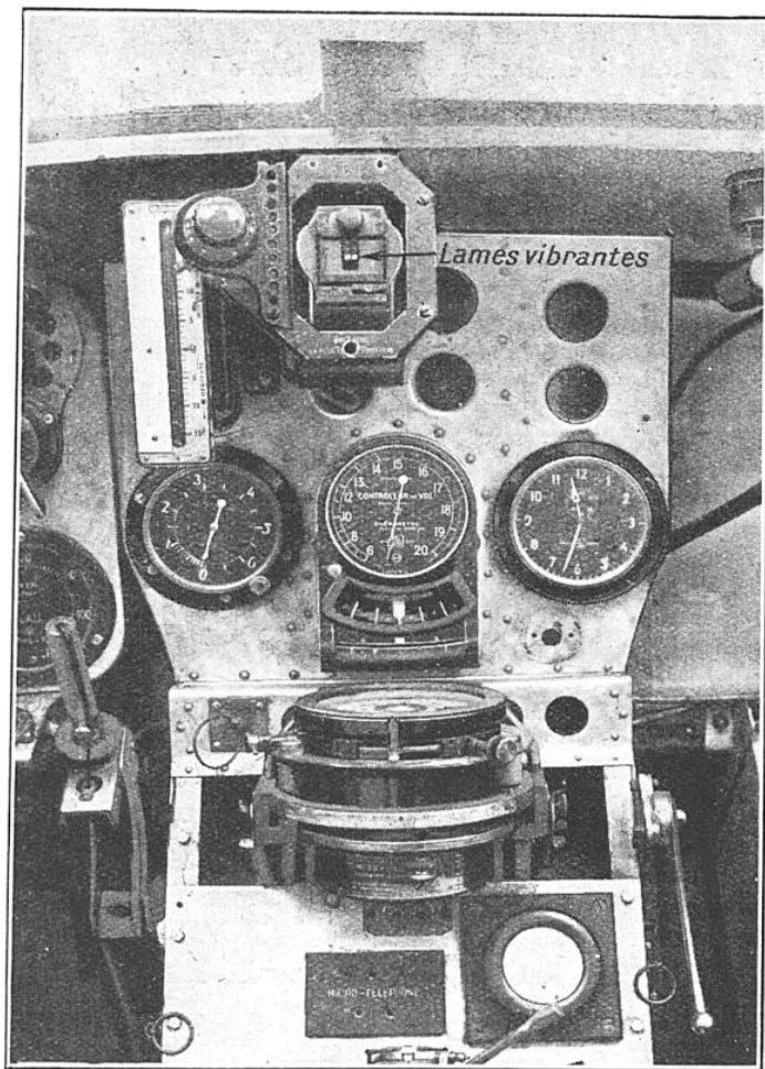
FIG. 10. — EMBLACEMENT DE L'INDICATEUR DE POSITION SUR UN AVION DE L'« AIR-UNION »
