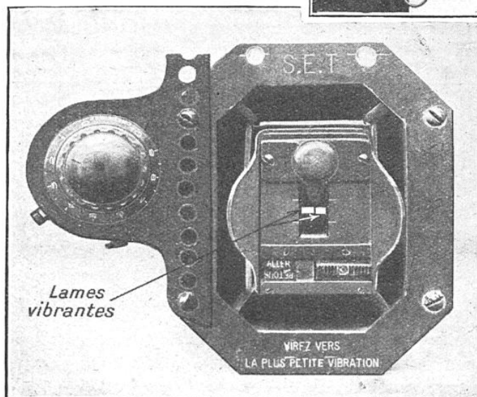
FIG. 9. — VUE DE FACE DE L'INDICATEUR DE POSITION SITUÉ DEVANT LE PILOTE, SUR LE TABLEAU DE BORD
