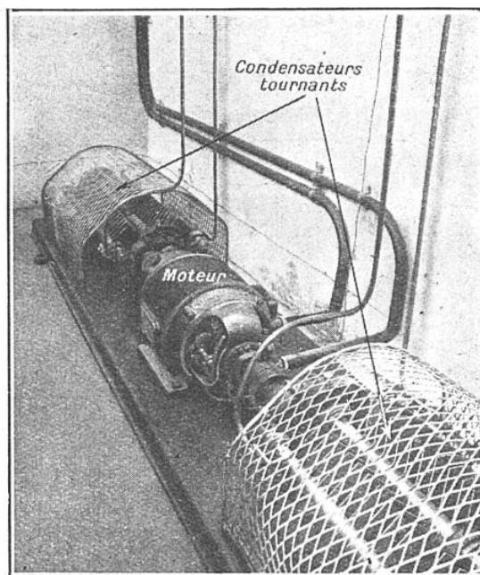
FIG. 7. — LES CONDENSATEURS TOURNANTS QUI AGISSENT SUR LES CIRCUITS DU NOUVEAU RADIOPHARE DU BOURGET
