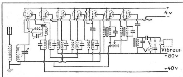
FIG. 6. — SCHÉMA DU RÉCEPTEUR INSTALLÉ SUR L'AVION
