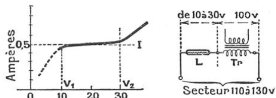
FIG. 7. — CARACTÉRISTIQUE DE LA LAMPE À HYDROGÈNE ET SON MONTAGE POUR LA RÉGULARISATION DE LA TENSION D'ALIMENTATION DU POSTE
