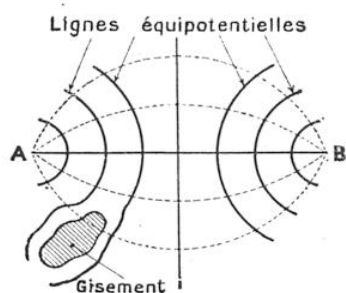
FIG. 2. — LES MÉTHODES ÉLECTRIQUES PERMETTENT DE DÉCELER LES GISEMENTS. Les mesures de résistivité du sol effectuées entre A et B servent à établir les lignes équipotentielles. Les irrégularités dans ces lignes indiquent la présence de gisements.
