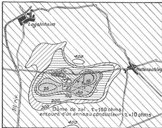
FIG. 9. — LE SONDAGE ÉLECTRIQUE PERMET DE DÉCELER LES DOMES DE SEL.
