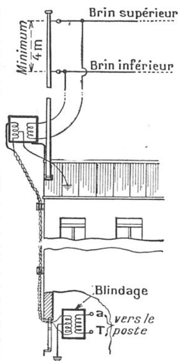
FIG. 10. — AUTRE DISPOSITIF POUR DIMINUER L'ACTION DES PARASITES ATMOSPHÉRIQUES
