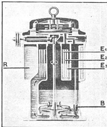
FIG. 3. RHÉOSTAT EN PÉRIODE DE DÉMARRAGE. Moteur et turbine sont en rotation depuis un certain temps déjà. Les électrodes médianes E 1 , E 2 , E 3 sont de plus en plus noyées. La résistance électrique diminue, le moteur
