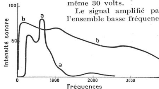
FIG. 20. — COURBE DE « RÉPONSE » DE HAUT-PARLEURS ANCIEN ET MODERNE
