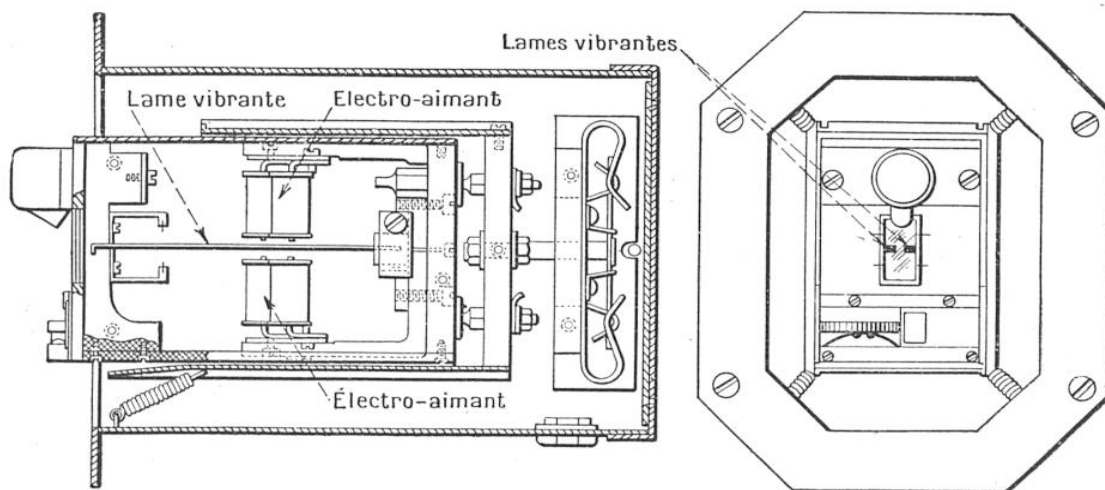
FIG. 5. — VUE, EN COUPE ET DE FACE, DE L'APPAREIL PLACÉ SUR L'AVION ET INDICANT AU PILOTE SA POSITION PAR RAPPORT A L'AXE DE BALISAGE
