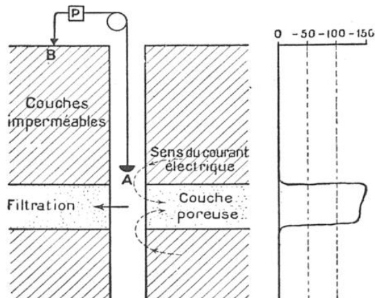
FIG. 7. — COMMENT LA PROSPECTION ÉLECTRIQUE PERMET DE DÉCELER UNE COUCHE POREUSE DANS UN FORAGE
