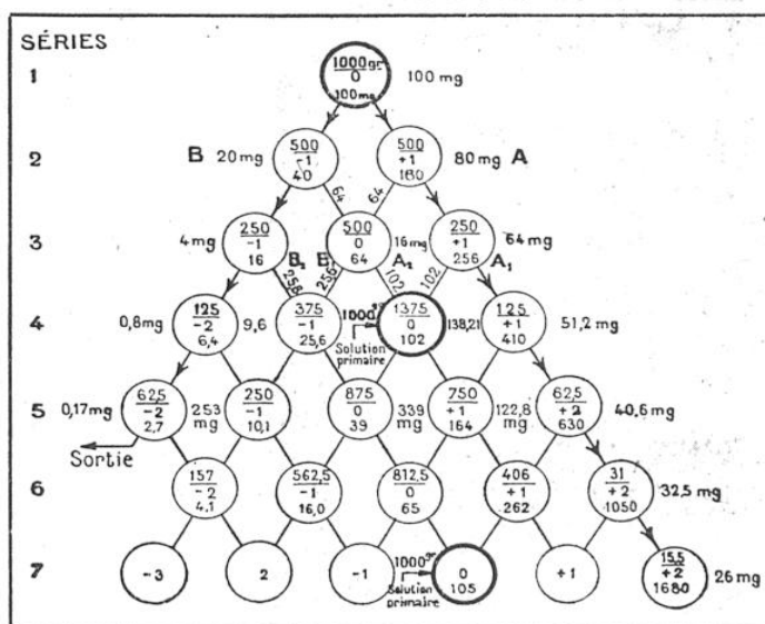
FIG. 4. — SCHÉMA DES SÉRIES SUCCESSIVES DE CRISTALLISATIONS FRACTIONNÉES D'UNE SOLUTION RADIFÈRE. Le schéma ci-dessus traduit, à partir d'une solution initiale (cercle en trait gras), la marche de la cristallisation effectuée sur les chlorures mélangés (et qu'il s'agit de séparer) de Baryum et de Radium. Le point de départ étant 1 kilogramme de sels contenant 100 milligrammes de Radium, l'opération consiste à diviser (par cristallisations et décantations successives) la masse cristalline totale en deux parties égales, dont l'une, la plus pauvre en Radium, reste dissoute dans l'eau mère, et l'autre, la plus riche, est séparée à l'état anhydre. Par cette dichotomie, prolongée en autant de subdivisions qu'il le faut, on aboutit à un degré de concentration des eaux mères égale à la concentration primitive, et c'est le cas indiqué par un nouveau cercle en trait gras (4 e série). A ce degré, l'on ajoute de la solution primitive et l'on continue à subdiviser, tandis que les sels anhydres séparés sont traités à nouveau, de la même façon, après nouvelle dissolution en eau distillée. Chaque cercle représente un état de dissolution : les cercles marqués d'un numéro négatif représentent les eaux mères ; les cercles numérotés positivement représentent les solutions concentrées. Le premier nombre inscrit en tête du cercle indique la masse totale des sels en solution ; le nombre inscrit à la base indique la teneur en Radium. Le nombre de milligrammes de chlorure de Radium « anhydre » entraîné dans la cristallisation est inscrit hors du cercle. On voit ainsi que les 100 milligrammes initiaux se concentrent de plus en plus dans les solutions de droite, d'où on extraira le Radium, tandis que les solutions de gauche s'appauvrissent, au contraire, indéfiniment.
