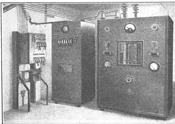
FIG. 8. — L'ÉMETTEUR DU RADIOPHARE DU BOURGET
