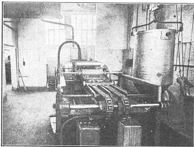
FIG. 8. — L'« OVOMALTINE » DESSÉCHÉE EST RÉDUITE EN FINES PAILLETTES. ELLE EST EMPORTÉE ALORS DANS LA TRÉMIE, A DROITE, VERS L'ATELIER D'ENSACHAGE
