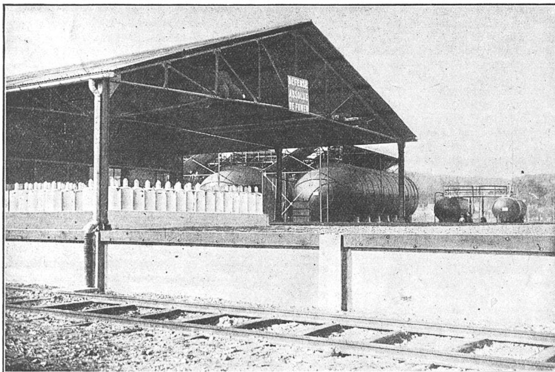
FIG. 6. — STOCKAGE DU BUTANE A L'USINE DE PETIT-COURONNE, PRÈS DE ROUEN
