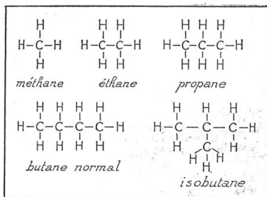
FIG. 1. — FORMULES DÉVELOPPÉES DES « PARAFFINES » LES PLUS SIMPLES, MONTRANT LA SATURATION DE TOUTES LES VALENCES
