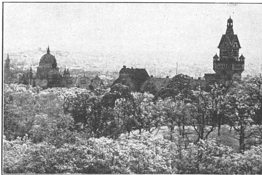
FIG. 5. — LA MÊME PHOTOGRAPHIE PRISE AVEC UNE PLAQUE SPÉCIALE SENSIBILISÉE AUX RAYONS INFRAROUGES (PHOTO « AGFA »). Les arrière-plans sont nettement visibles. Les premiers plans (verdure) sont blancs et donnent un effet de neige (effet de Wood).
