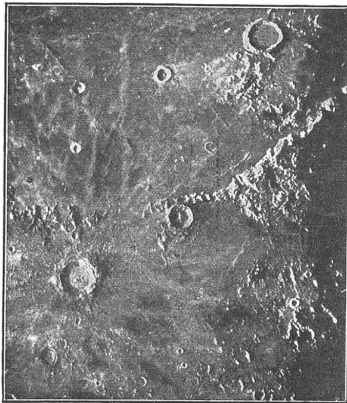
FIG. 7 — VOICI UN FRAGMENT DE LA SURFACE DE LA LUNE (RÉGION DE COPERNIC)
