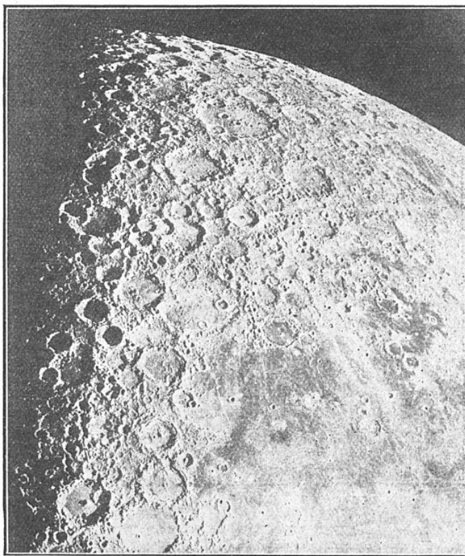
FIG. 6. — PHOTOGRAPHIE DE LA SURFACE DE LA LUNE La surface de la Lune est couverte de grands cratères.
