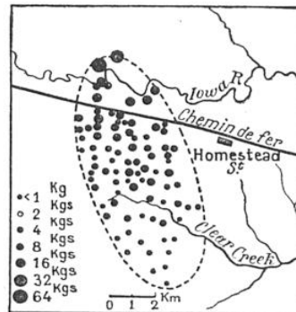
FIG. 1. — RÉPARTITION DES MÉTÉORITES, A LA SUITE D'UNE GRÊLE DE PIERRES QUI EUT LIEU, EN 1875, A HOMESTEAD (IOWA)
