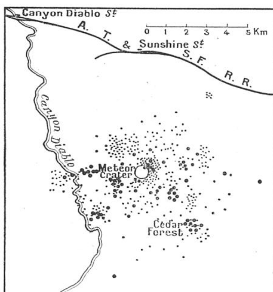
FIG. 4. — DISTRIBUTION DES FRAGMENTS DE MÉTÉORITES AUTOUR DU METEOR CRATER Tous les fragments recueillis sont extérieurs au cirque représenté ci-dessus, mais sans en être éloignés de plus de 9 kilomètres.
