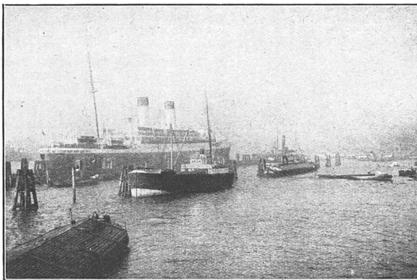
FIG. 7. — VUE DU MÊME PORT, PRISE AVEC UNE PLAQUE ORDINAIRE
