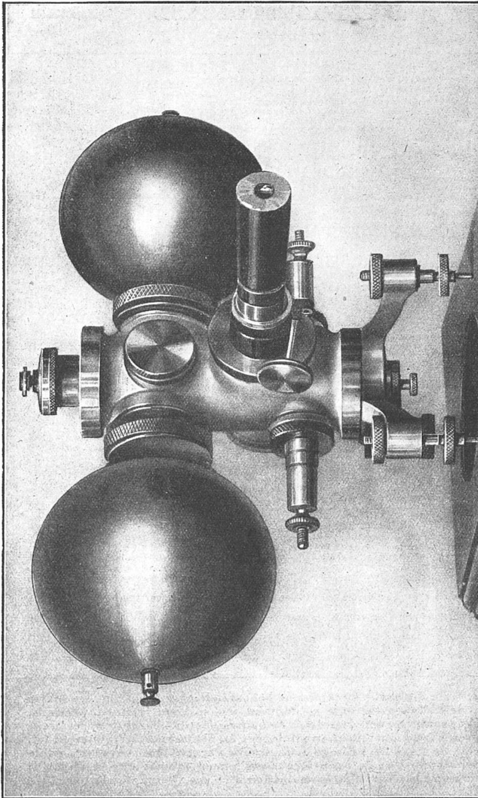
L'ÉLECTROMÈTRE « COMPENSÉ » QUI SERT, AU LABORATOIRE DE L'USINE D'OOLEM PRÈS D'ANVERS (BELGIQUE), À MESURER, D'UNE FAÇON PRÉCISE, LA RADIOACTIVITÉ DU MINÉRAI D'URANIUM-RADIUM AUX DIFFÉRENTS STADES DE SA CONCENTRATION. Chacune des deux sphères représente une « chambre d'ionisation », au centre de laquelle est une électrode. L'électromètre (dont la lecture se fait par visée dans l'oculaire central visible au milieu de l'appareil) est monté en « différentiel » sur les deux électrodes. Au moment de la mesure, l'une des chambres est masquée par un écran de plomb, tandis que l'autre est exposée au rayonnement du corps radioactif.
