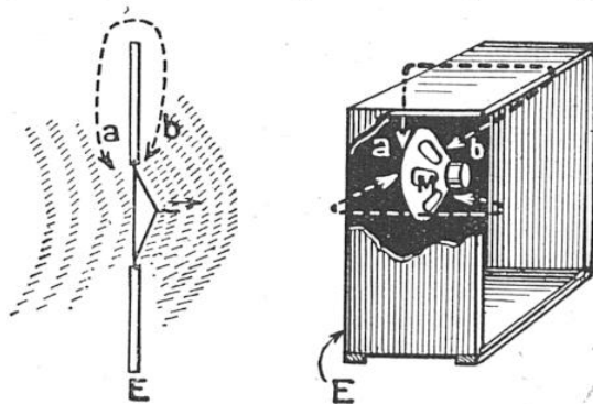
FIG. 22. — ON ÉVITE LE « COURT-CIRCUIT ACOUSTIQUE » AU MOYEN D'UN ÉCRAN E, DE SORTE QUE LE TRAJET ENTRE a ET b EST SUFFISAMMENT LONG POUR ÉVITER LE PHÉNOMÈNE INDICÉ FIGURE 21
