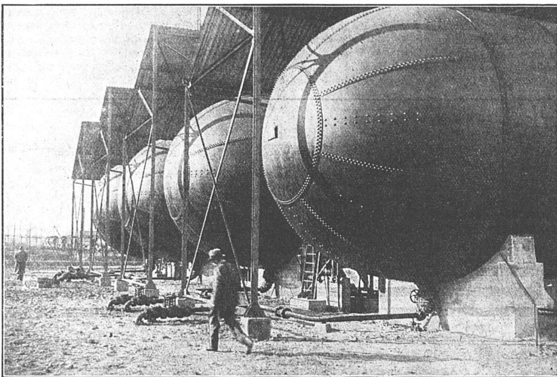
FIG. 5. — VUE AVANT DES QUATRE RÉSERVOIRS PRINCIPAUX DE PETIT-COURONNE, PRÈS ROUEN
