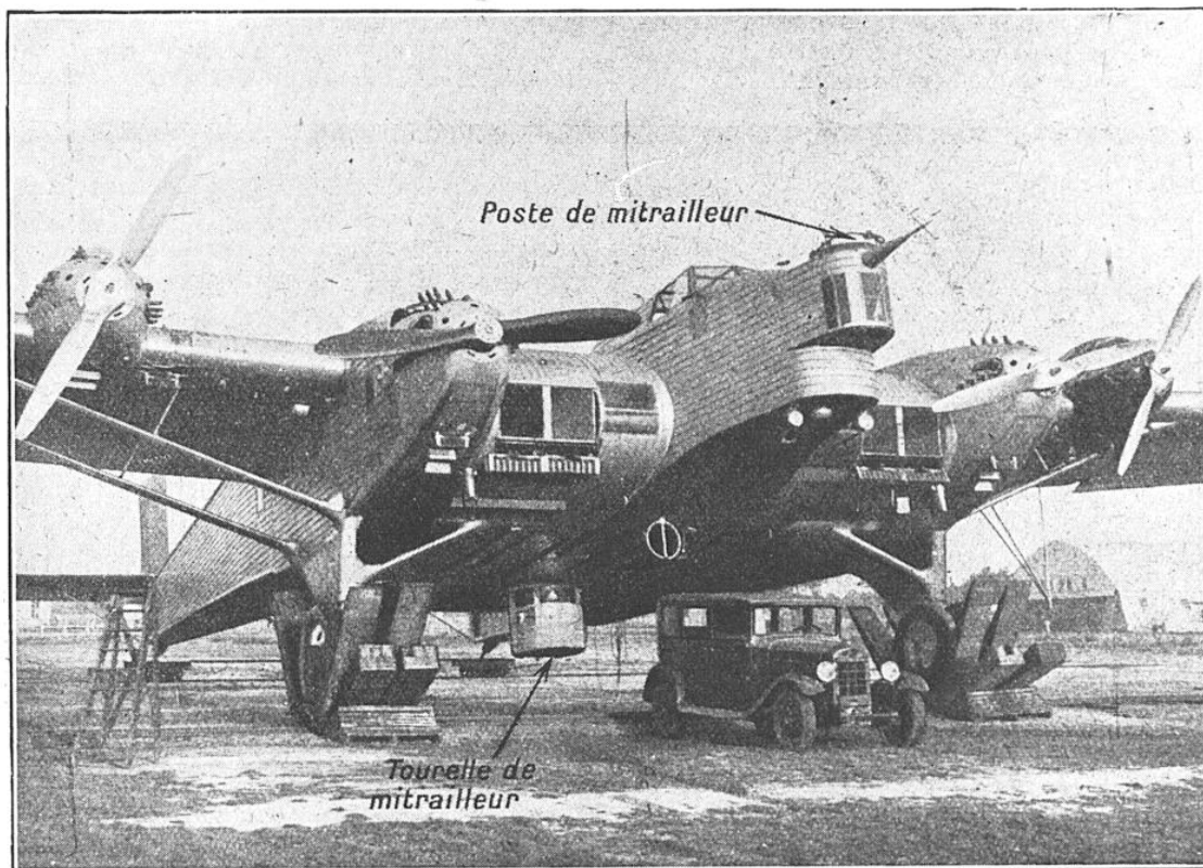
FIG. 6. — L'AVION GÉANT FRANÇAIS DE BOMBARDEMENT « S. A. B. 70 » Cet avion, à deux fuselages, de 37 mètres d'envergure et de 21 m 40 de long, est muni de quatre moteurs dont la puissance totale atteint 2.040 ch. La vitesse de l'appareil est de 215 km/heure.
