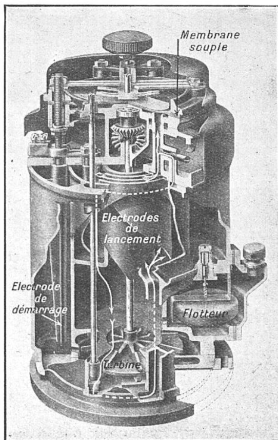
FIG. 1. — VUE D'ENSEMBLE DU DÉMARREUR POUR MOTEUR ÉLECTRIQUE DE M. PLANCHE, MONTRANT SES DIFFÉRENTS ORGANES
