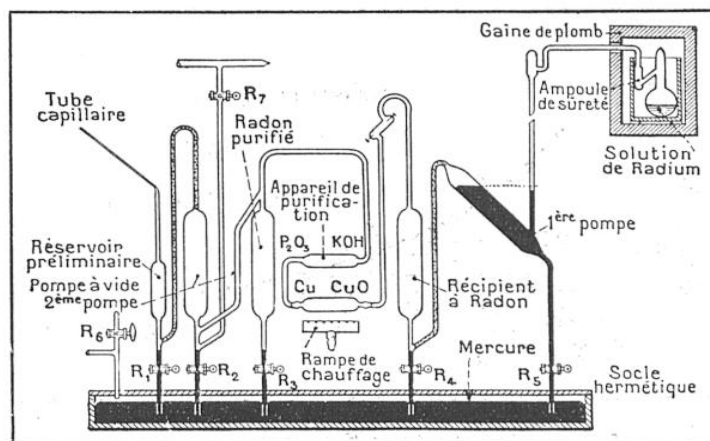
FIG. 10. — SCHÉMA D'UN APPAREIL SERVANT À L'EXTRACTION DU « RADON » ÉMANATION DU RADIUM
