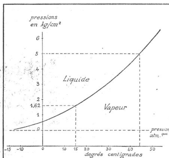
FIG. 2. — VARIATIONS DE LA PRESSION MAXIMUM DU BUTANE COMMERCIAL EN FONCTION DE LA TEMPÉRATURE
