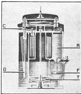
FIG. 2. RHÉOSTAT AU REPOS, PRÊT À DÉMARRER. Moteur à l'arrêt ou sur première phase de démarrage (mise en route de la turbine T, qui, commençant seulement à tourner, ne produit pas encore de pression appréciable). L'électrolyte est au
