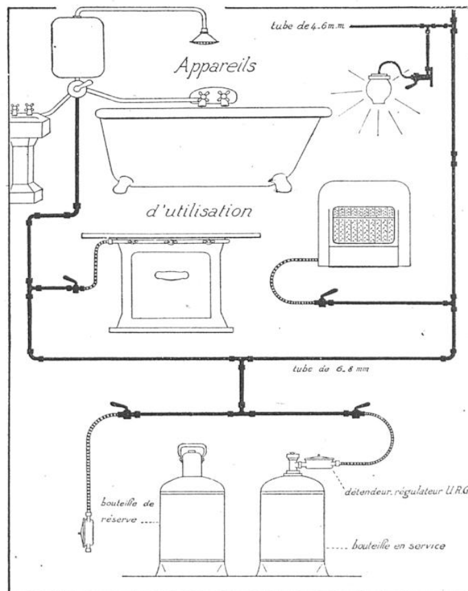
FIG. 10. — SCHÉMA D'UN DOUBLE POSTE « U. R. G. » ET DE L'INSTALLATION DE QUELQUES APPAREILS D'UTILISATION
