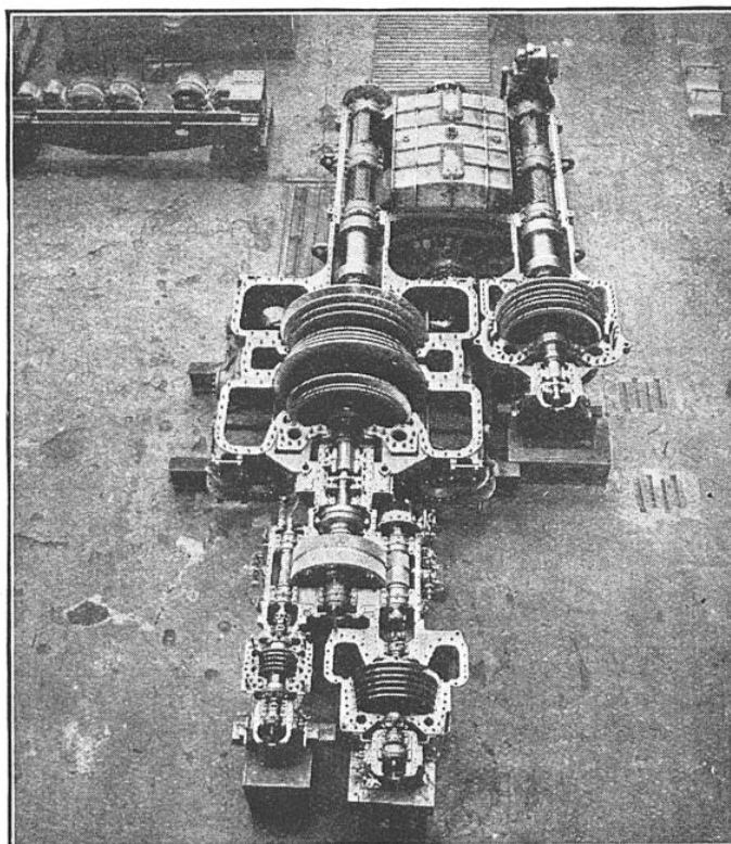
FIG. 4. — ENSEMBLE D'UN DES DEUX GROUPES MOTEURS DU CONTRE-TORPILLEUR « CASSARD »
