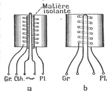
FIG. 3. — SCHÉMA D'UN FILAMENT DE LAMPE DE T. S. F. A CHAUFFAGE INDIRECT (A GAUCHE) ET A CHAUFFAGE DIRECT (A DROITE)
