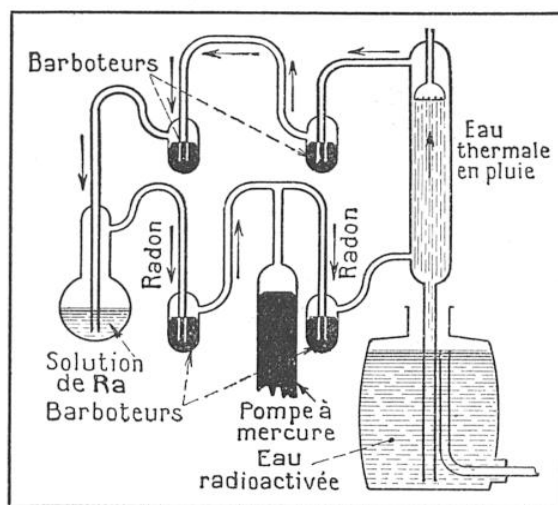
FIG. 13. — APPAREIL A « RADIOACTIVER » L'EAU PAR DISSOLUTION DE RADON
