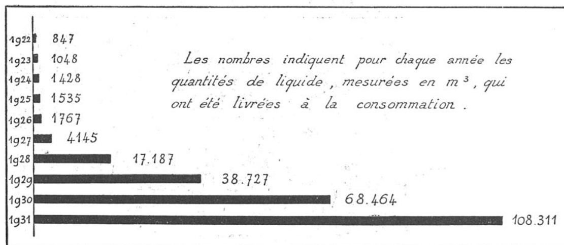
FIG. 3. — ESSOR DE L'INDUSTRIE DES GAZ DE PÉTROLE LIQUÉFIÉS (BUTANE ET PROPANE) AUX ÉTATS-UNIS, AU COURS DES DIX DERNIÈRES ANNÉES
