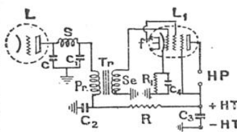
FIG. 16 ET 17. — AMPLIFICATEURS BASSE FRÉQUENCE À LIAISON ENTRE ÉTAGES, PAR TRANSFORMATEURS (A GAUCHE) ET PAR RÉISTANCES (A DROITE)
