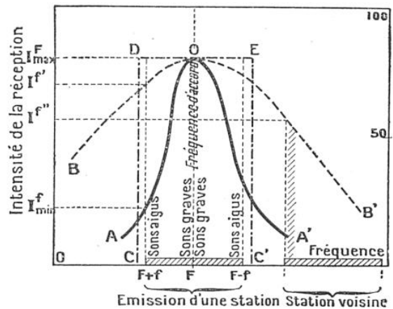
FIG. 12. — DIVERSES FORMES DES COURBES DE RÉSONANCE D'UN CIRCUIT ACCORDÉ
