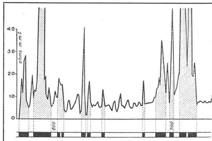
FIG. 12. — LE « CAROTTAGE » ÉLECTRIQUE A DONNÉ D'INTÉRESSANTS RÉSULTATS POUR LA RECHERCHE DES CHAMPS PÉTROLIFÈRES EN AMÉRIQUE DU SUD
