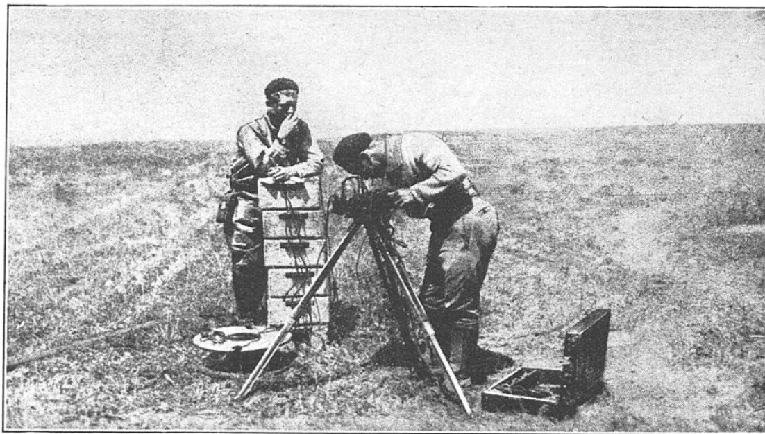
FIG. 11. — PROSPECTION ÉLECTRIQUE RÉALISÉE DANS LA PLAINE DU TEREK (U. R. S. S.)
