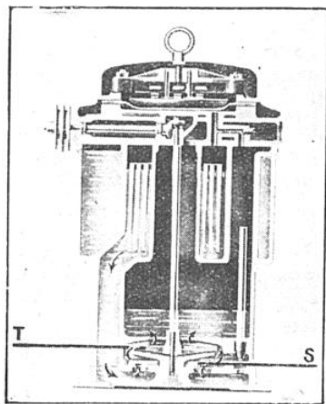
FIG. 6. RHÉOSTAT VENANT DE S'ARRÊTER MONTRANT LE RETOUR RAPIDE DU LIQUIDE
