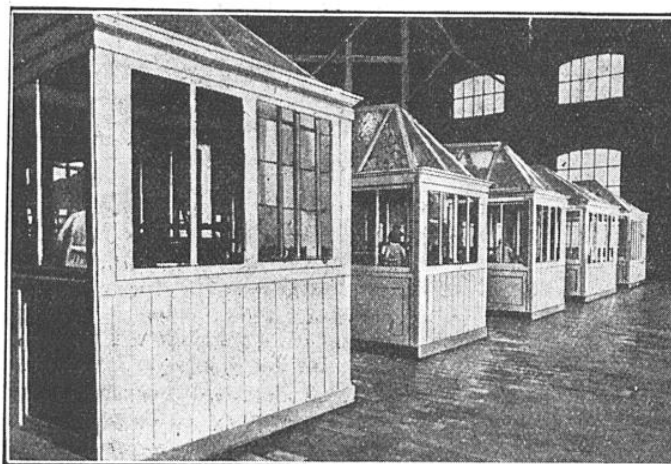
FIG. 3. — LES CABINES-ABRIS OU S'EFFECTUENT LES CRISTALLISATIONS FRACTIONNÉES AU BOUT DESQUELLES LE RADIUM EST ISOLÉ A L'ÉTAT DE CHLORURE
