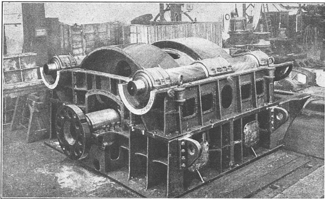
FIG. 2. — LE TRAIN D'ENGRENAGES RÉDUCTEURS INTERPOSÉ ENTRE CHAQUE TURBINE ET L'HÉLICE QU'ELLE COMMANDE SUR LE CONTRE-TORPILLEUR « CASSARD »
