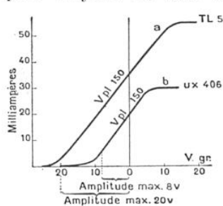
FIG. 19. — COURBES D'AMPLIFICATION DE LAMPES A BASSE FRÉQUENCE
