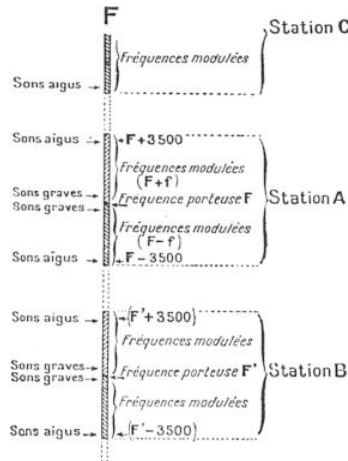
FIG. 11. — COMMENT SE PRÉSENTENT LES BANDES DE FRÉQUENCES ÉMISES PAR TROIS STATIONS VOISINES A, B, C
