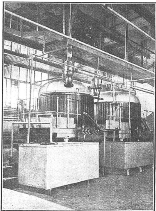
FIG. 5. — CUVES OU SE PRÉPARE L'INFUSION DU GRAIN MALTÉ DANS DE L'EAU A 50°
