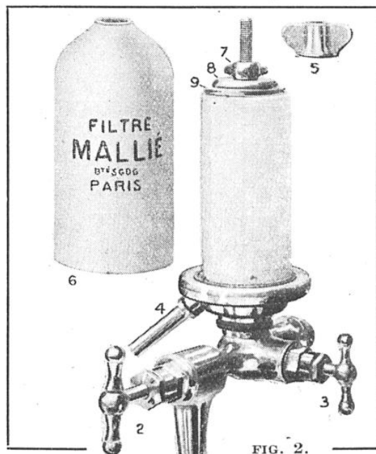
LE FILTRE DÉMONTÉ POUR NETTOYAGE
