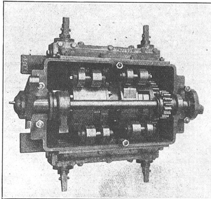
FIG. 7. — VUE D'UN TAMBOUR DE DISTRIBUTION DE LA « MOUNTAIN » DE L'ÉTAT, MONTRANT LES COULISSEAUX ET LES GALETS PORTÉS PAR L'EXTRÉMITÉ DES CULBUTEURS ACTIONNANT LES TIGES DE SOUPAPES
