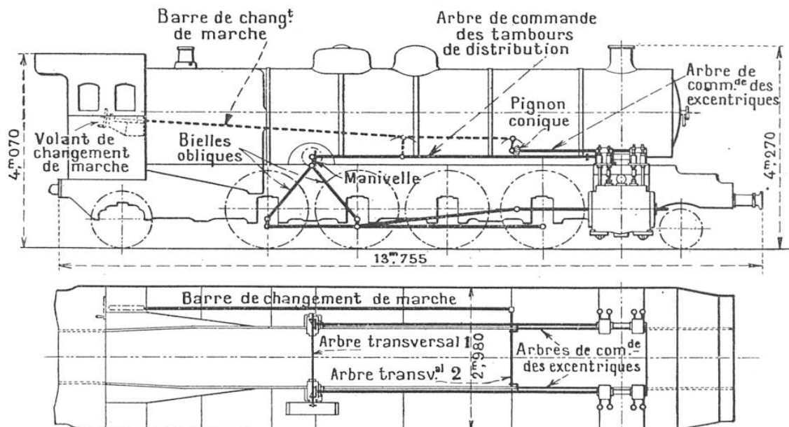
FIG. 6. — ENSEMBLE D'UNE DISTRIBUTION DE VAPEUR PAR SOUPAPES, SYSTÈME RENAUD, MONTÉ SUR UNE LOCOMOTIVE « MIKADO » DE L'ÉTAT
