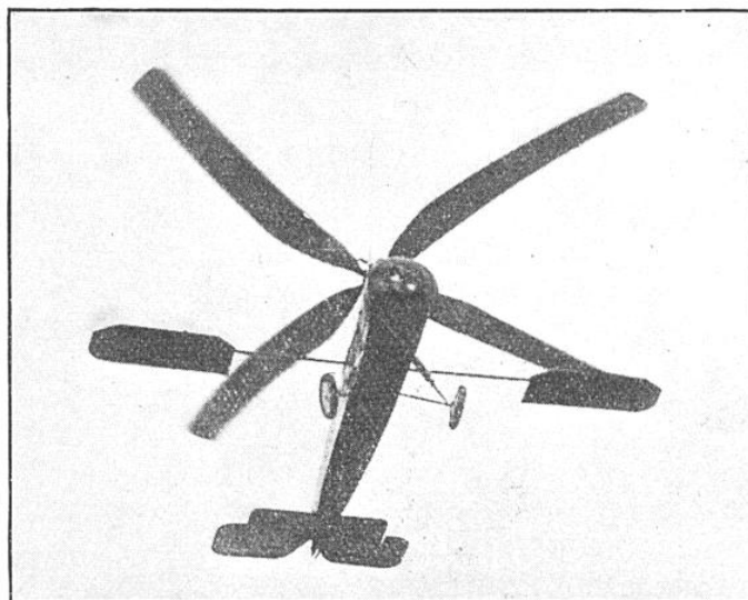
FIG. 8. — LE PREMIER AUTOGIRE A ROTOR ARTICULÉ EN PLEIN VOL. IL COMPORTAIT DEUX PLANS LATÉRAUX
