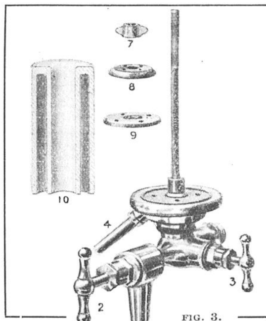
LE FILTRE COMPLÈTEMENT DÉMONTÉ
