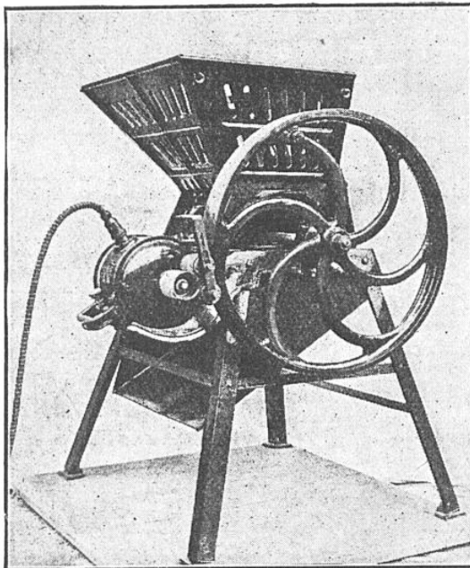
FIG. 3. — APPAREIL COUPE-RACINES MUNI DE SON MOTEUR PORTATIF. POUR DE TELS APPAREILS, LA PUISSANCE EST ASSEZ FAIBLE ; ELLE OSCILLE ENTRE 1, 2 ET 3 CHEVAUX, SELON LE DÉBIT QUE L'ON DÉSIRE
