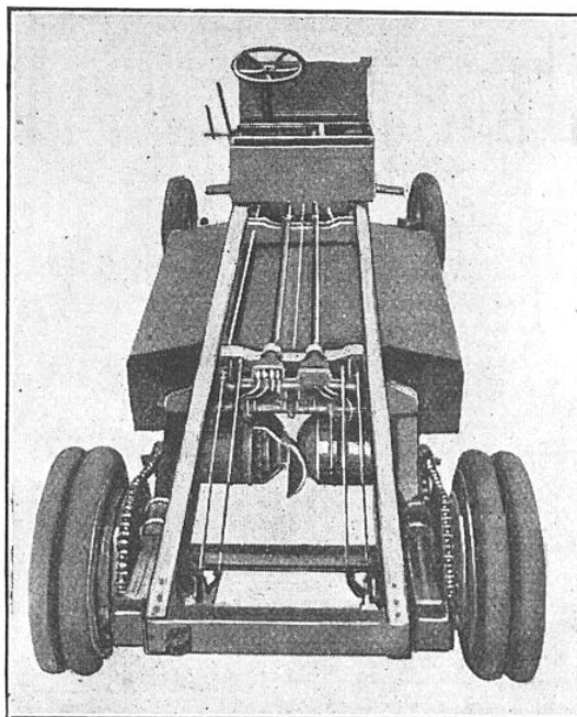
FIG. 2. — CHASSIS ÉLECTRIQUE
