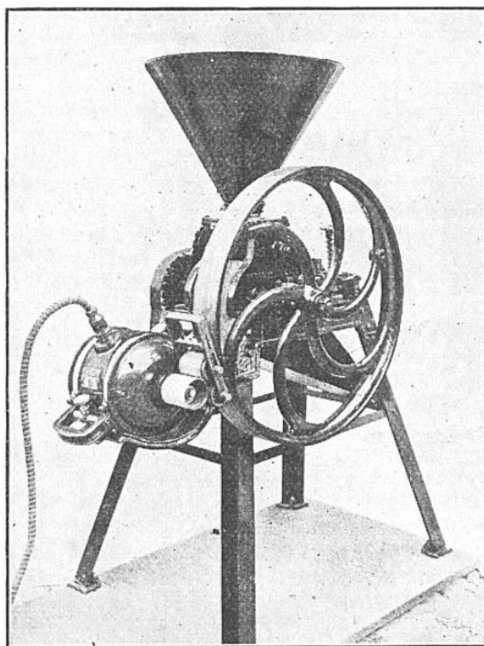
FIG. 4. — APLATISSEUR DE GRAINS ÉGALEMENT MUNI D'UN MOTEUR PORTATIF
