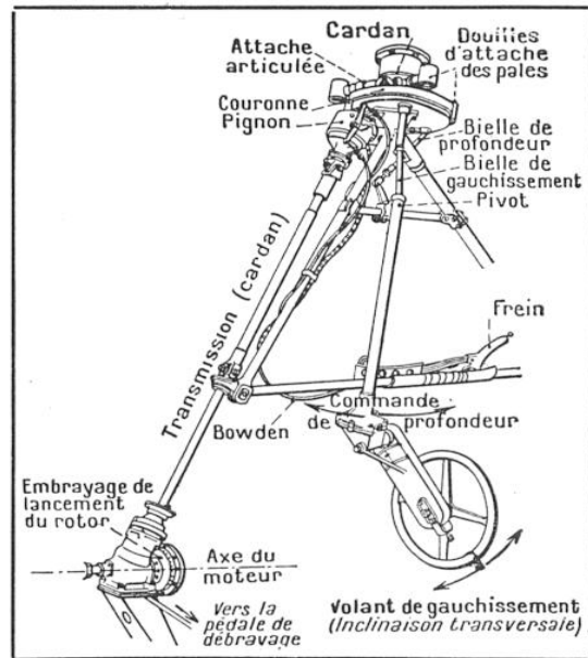
FIG. 12. — ENSEMBLE DES COMMANDES DANS L'AUTOGIRE « C.-L. 10 »
