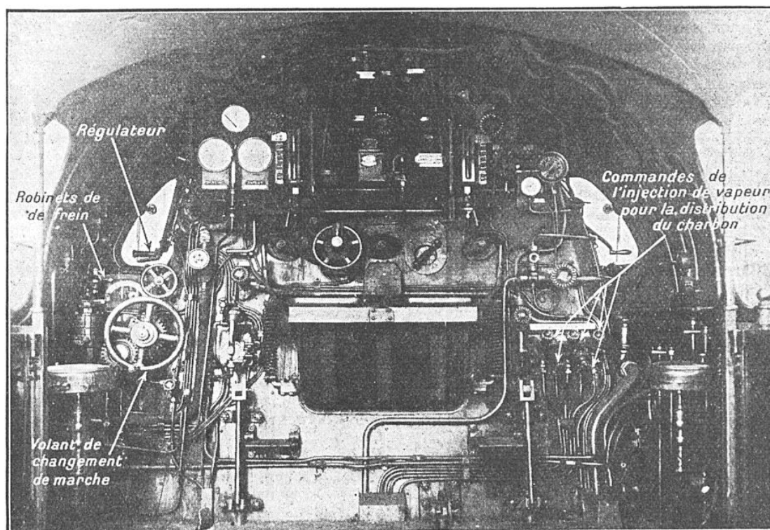
FIG. 8. — ENSEMBLE DE L'ABRI DU MÉCANICIEN DE LA LOCOMOTIVE « MOUNTAIN » DE L'ÉTAT
