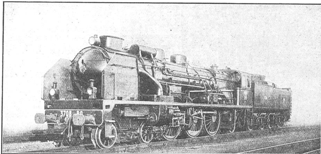
FIG. 10. — UNE DES NOUVELLES « PACIFIC » DU P.-O., DE LA SÉRIE 3700, DONT LA PUISSANCE RIVALISE AVEC CELLE DES « MOUNTAIN »
