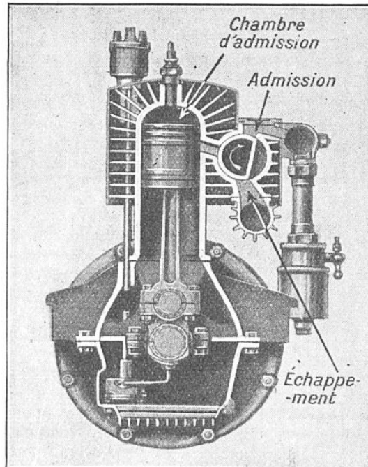
FIG. 1. — UN MOTEUR SANS SOUPAPES ET SANS EAU DE REFROIDISSEMENT
