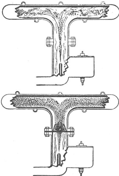
COMMENT SE PRODUIT LE MÉLANGE AIR-ESSENCE : EN HAUT, SANS TURBO-DIFFUSEUR ; EN BAS, AVEC TURBO-DIFFUSEUR
