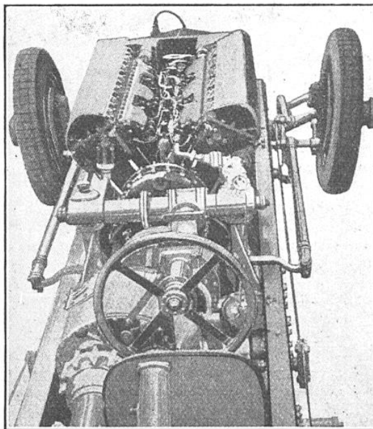
FIG. 1. — LE CHASSIS DE L'« OISEAU-BLEU » A l'avant, on voit le moteur Rolls Royce de 12 cylindres. On remarquera que le siège du conducteur est décalé vers la droite pour permettre, sur la gauche, le passage de l'arbre de transmission.
