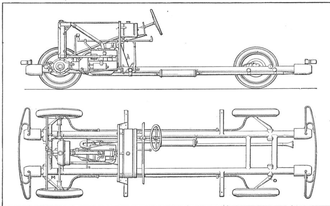
FIG. 5. — CHASSIS A ROUES INDÉPENDANTES ET TRACTION PAR L'AVANT
