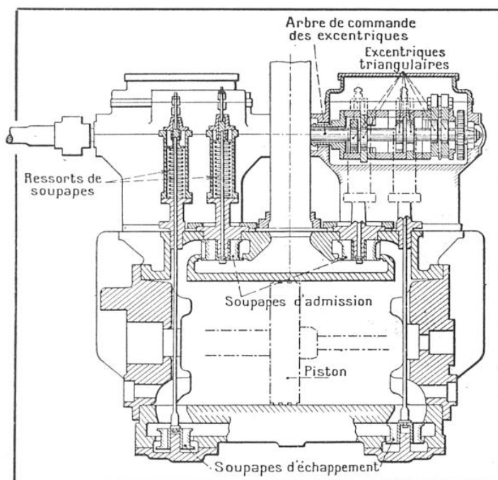
FIG. 3. — COUPE D'UN CYLINDRE DE LA « MOUNTAIN » DE L'ÉTAT, MONTRANT LES SOUPAPES D'ADMISSION ET D'ÉCHAPPEMENT, AVEC LEUR DISPOSITIF DE COMMANDE
