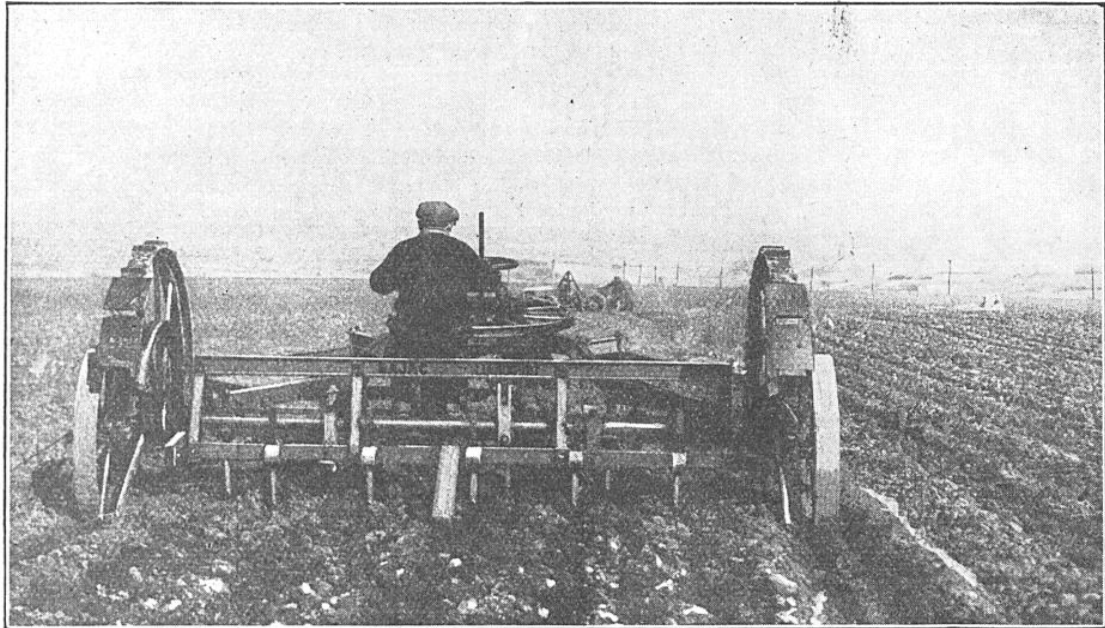
FIG. 1. — VOICI UN SCARIFICATEUR MU PAR UN TREUIL ÉLECTRIQUE. LA LARGEUR DU TERRAIN TRAVAILLÉ PAR CET APPAREIL, QUI AMEUBLIT LA TERRE, EST DE 3 M 50
