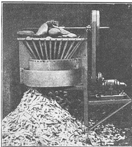
FIG. 2. — TRANSPORTABLE A BRAS, UN PETIT MOTEUR ÉLECTRIQUE PLACÉ DANS UN BERCEAU SPÉCIALEMENT AMÉNAGÉ SUR LE BÂTI DE CETTE MACHINE PERMET DE DÉBITER 2 TONNES DE BETTERAVES EN 45 MINUTES, POUR UN PRIX INFÉRIEUR A 1 FRANC
