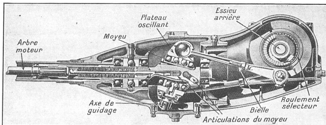
FIG. 3. — CHANGEMENT DE VITESSE AUTOMATIQUE SENSAUD DE LAVAUD
