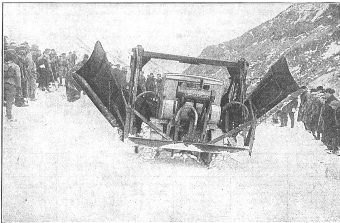
FIG. 2. — LES AILERONS ARRIÈRE D'UN CHASSE-NEIGE A ÉTRAVE SONT UTILISÉS POUR ÉLARGIR LA VOIE TRACÉE PAR L'ÉTRAVE ET REJETER LA NEIGE DE CHAQUE COTÉ DE LA ROUTE
