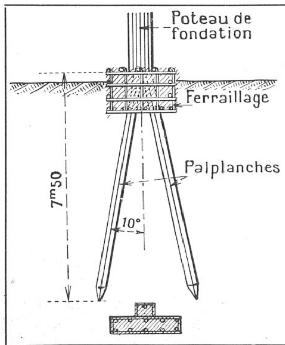
FIG. 9. — UN ÉLÉMENT DES FONDATIONS DU BUILDING-HOPITAL
