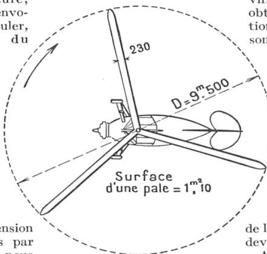
FIG. 10. — VUE EN PLAN DE L'AUTOGIRE « C.-L. 10 »
