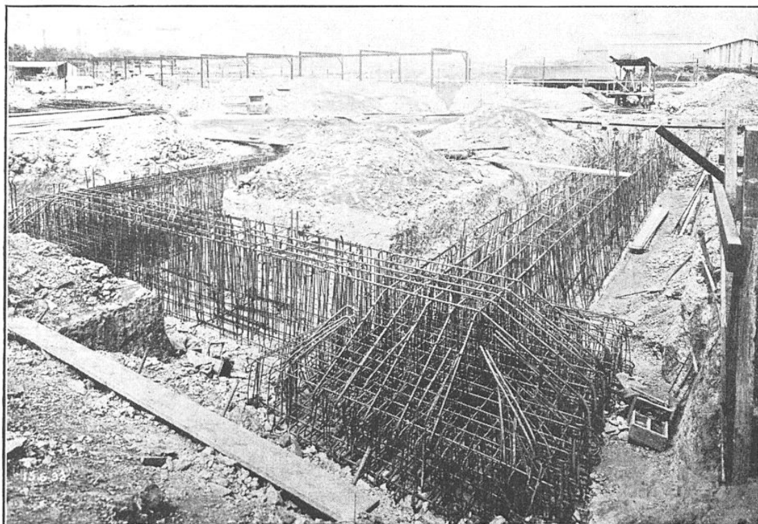
FIG. 10. — LE FERRAILAGE D'ENSEMBLE DES FONDATIONS D'UN CORPS DE BATIMENT
