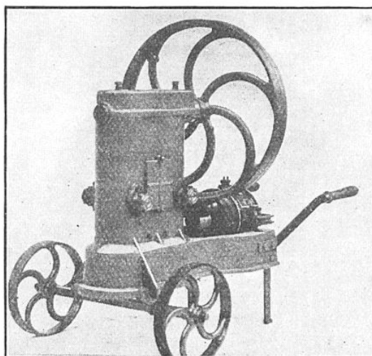
FIG. 7. — PETITE POMPE A MAIN MOBILE. SUR LE BÂTI DE LAQUELLE EST ÉGALEMENT MONTÉ UN MOTEUR PORTATIF
