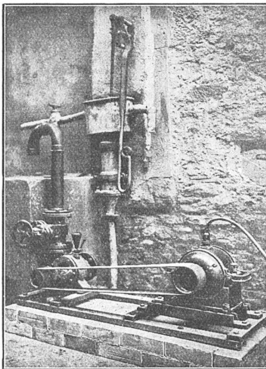
FIG. 8. — CETTE POMPE A MAIN A ÉTÉ REMPLACÉE PAR UN MOTEUR ÉLECTRIQUE Ce type de moteur est bien perfectionné. Il comporte un dispositif automatique permettant de couper le courant aussitôt que le réservoir servant à charger l'eau est plein.
