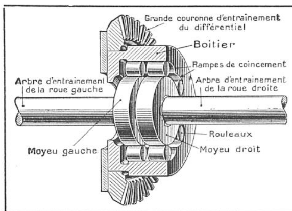
FIG. 4. — DIFFÉRENTIEL DE SÉCURITÉ ET ROUE LIBRE DE SAUSA DE LAVAUD
