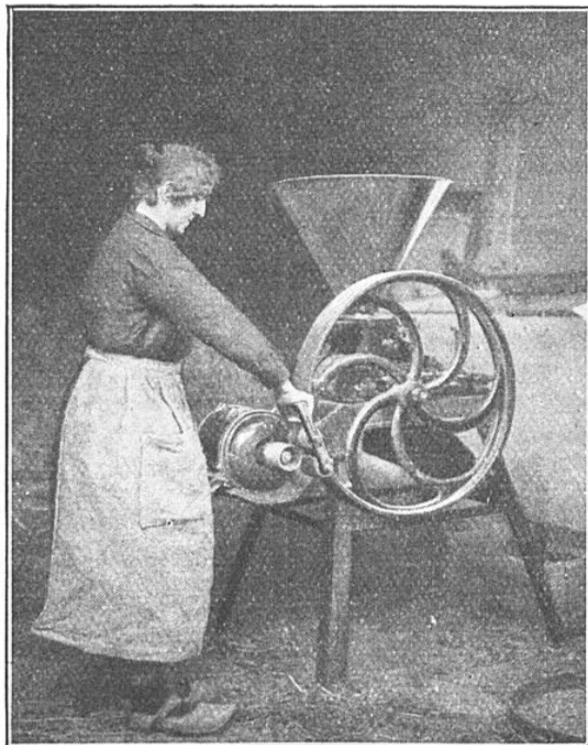
FIG. 6. — DEUXIÈME PHASE DU MONTAGE DE L'APLATISSEUR DE GRAINS DE LA FIGURE 5
