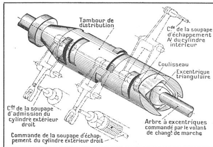
FIG. 5. — VUE EN PERSPECTIVE DU MÉCANISME DE COMMANDE DES SOUPAPES
