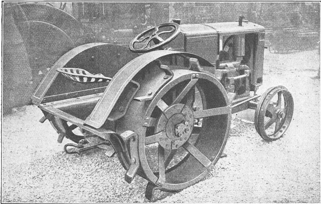
FIG. 2. — VOICI UN NOUVEAU TRACTEUR LÉGER DE FAIBLE PUISSANCE (8 CHEVAUX)
