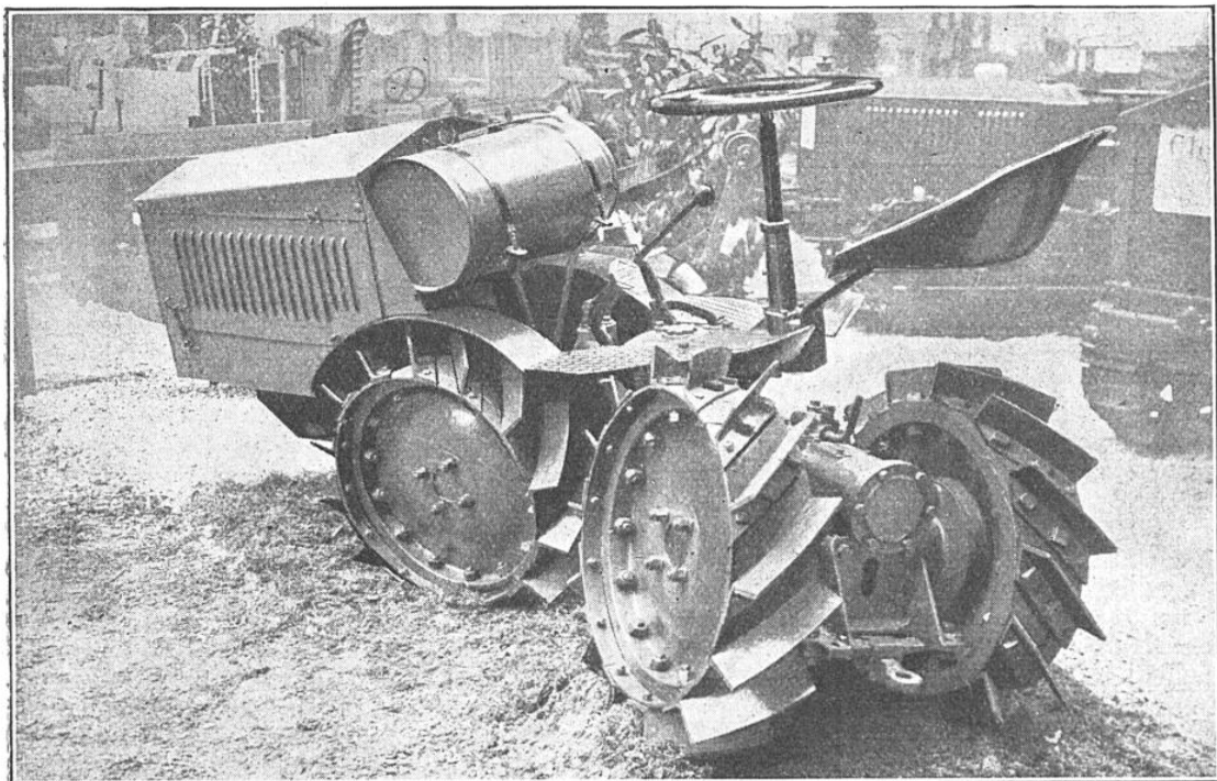
FIG. 3. — UN MODÈLE DE TRACTEUR ARTICULÉ A QUATRE ROUES MOTRICES ET DIRECTRICES POUVANT SE DÉPLACER DANS LES TERRAINS LES PLUS VARIÉS
