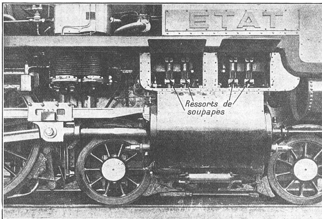
FIG. 2. — UN DES TROIS CYLINDRES DE LA « MOUNTAIN » DE L'ÉTAT. ON VOIT, AU-DESSUS DU CYLINDRE, LES TIGES ET LES RESSORTS DE SOUPAPES
