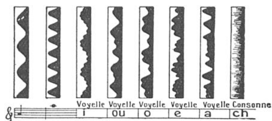
FIG. 2. — COMMENT S'ÉCRIVENT CERTAINS SONS, OU NOTES, SUR UNE BANDE SONORE
