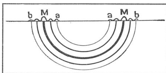
FIG. 5. — VOICI LA FORMATION D'UN TRAIN D'ONDES A LA SURFACE DE L'EAU
