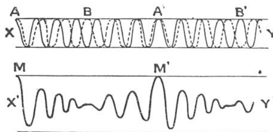
FIG. 4. — COMMENT LA COMPOSITION DES VIBRATIONS FORME LES TRAINS D'ONDES Les deux vibrations jaune et verte AB A'B' superposées le long du rayon lumineux X Y produisent un train d'ondes M M' le long de X' Y'.
