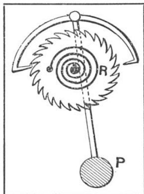
FIG. 3. — QU'EST-CE QU'UN « QUANTUM » D'ÉNERGIE ?
