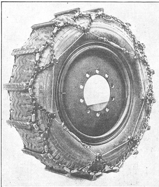
FIG. 10. — DISPOSITIF DE CHAÎNE UTILISÉ POUR DONNER L'ADHÉRENCE AUX ROUES DES TRACTEURS DE CHASSE-NEIGE. ON UTILISE AUSSI POUR CELA LES CHENILLES
