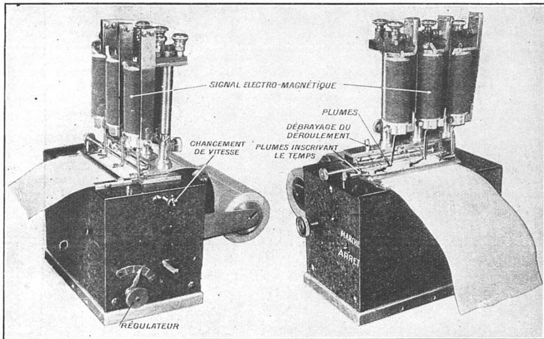
FIG. 9. — DISPOSITIF ENREGISTREUR-CHRONOMÈTRE UTILISÉ POUR LE CHRONOMÉTRAGE MÉCANIQUE DES ÉPREUVES D'ACCÉLÉRATION ET DE FREINAGE
