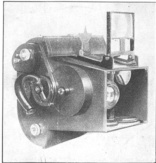
FIG. 2. — L'APPAREIL A MAIN DIT « ALTIPHOTE »
