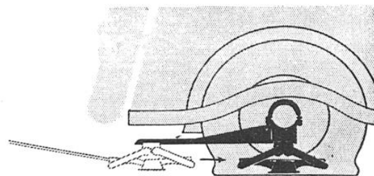
FIG. 5. — DEUX RAILS DE GUIDAGE PERMETTENT DE PLACER CORRECTEMENT LE CRIC SANS DIFFICULTÉ SOUS LA VOITURE
