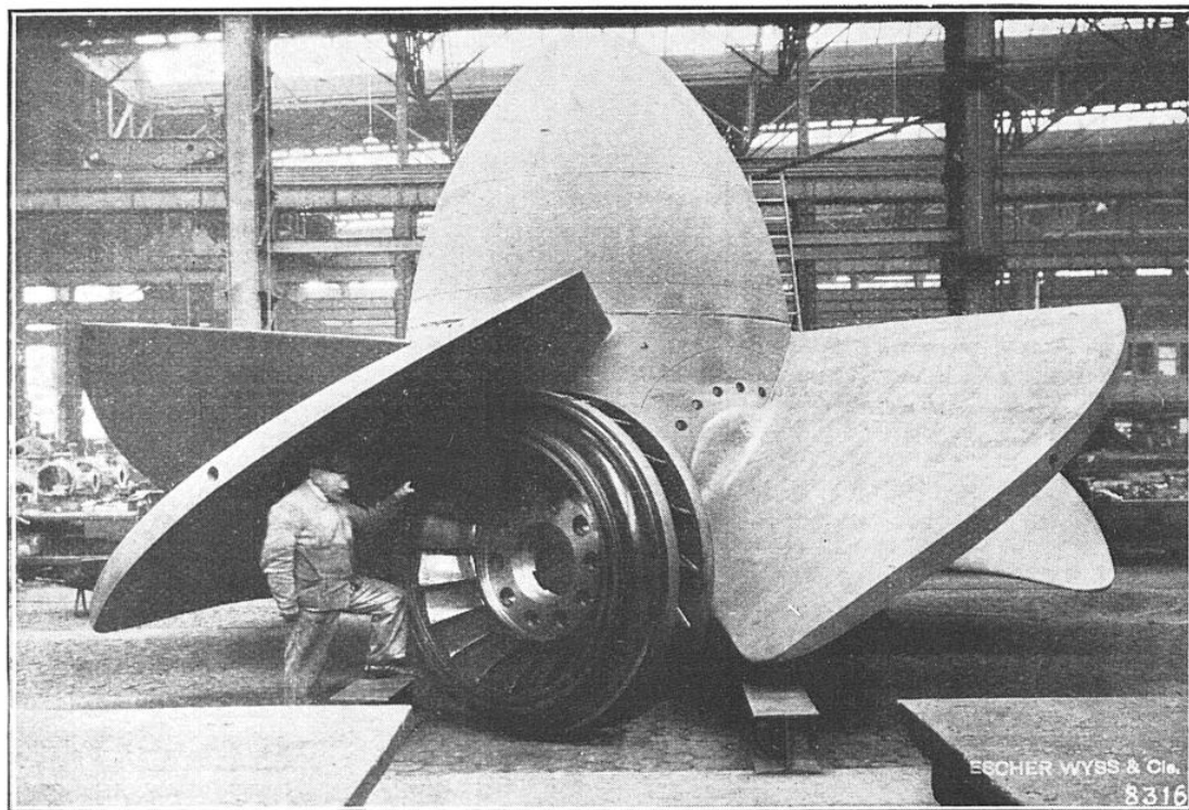
FIG. 4. — TURBINE « KAPLAN », DE 7 MÈTRES DE DIAMÈTRE, A CINQ AUBES MOBILES ORIENTABLES, UNE DES PLUS PUISSANTES DU MONDE A L'HEURE ACTUELLE
