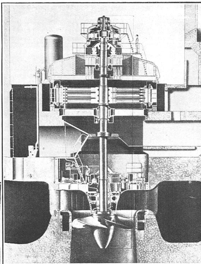
FIG. 6. — VUE EN COUPE D'UN DES GROUPES TURBOALTERNATEURS DE 36.600 CH DE LA CENTRALE DE KEMBS
