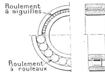
FIG. 9. — QUELLE EST LA DIFFÉRENCE D'ASPECT ENTRE UN ROULEMENT A AIGUILLES ET UN ROULEMENT A ROULEAUX ?
