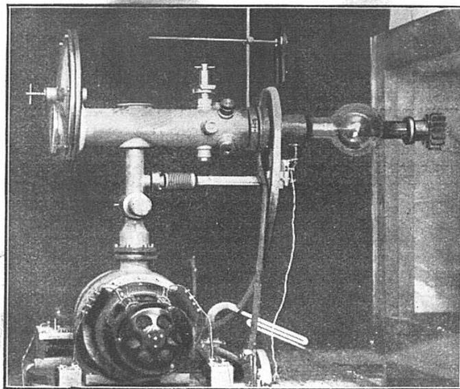
FIG. 4. — RÉALISATION D'UN APPAREIL POUR LA DIFFRACTION D'ÉLECTRONS RAPIDES (J.-J. TRILLAT)
