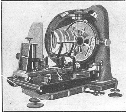
FIG. 12. — L'APPAREIL DE REDRESSEMENT QUI PERMET DE TRANSFORMER LES PHOTOS OBTENUES (FIG. 11) POUR OBTENIR UNE VUE D'ENSEMBLE TELLE QUE CELLE QUI EST REPRÉSENTÉE FIGURE 13
