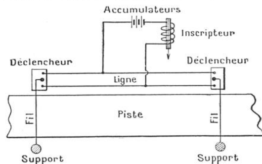
FIG. 6. — SCHÉMA D'ENSEMBLE D'UN DISPOSITIF MÉCANIQUE DE CHRONOMÉTRAGE
