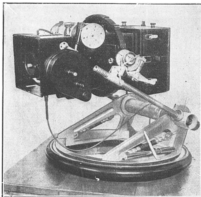
FIG. 9. — VOICI LE MÊME APPAREIL MUNI DE SON MAGASIN AUTOMATIQUE A PELLICULES
