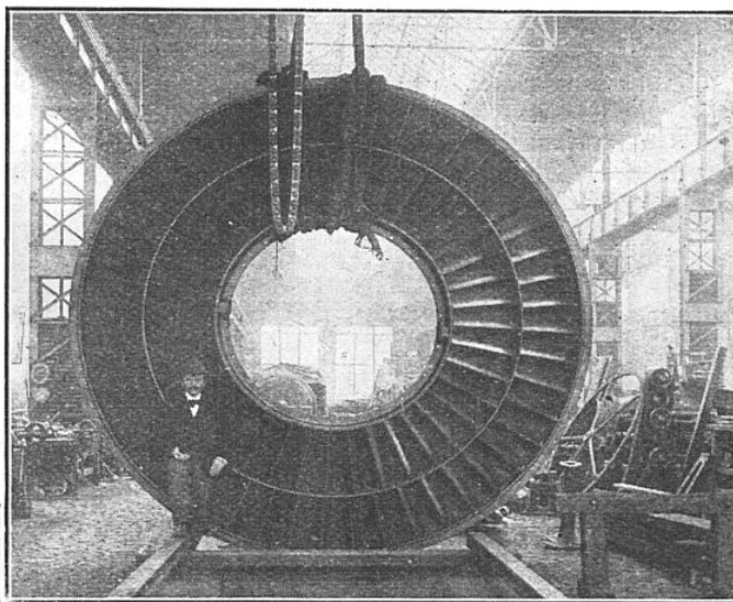
FIG. 3. — VOICI UNE ROUE DE TURBINE « JONVAL » DANS LAQUELLE LE MOUVEMENT DE L'EAU EST CONSTAMMENT AXIAL Ce type de turbine, qui date d'un siècle, ne tournait pas assez vite pour entraîner directement un alternateur.
