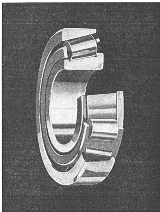
FIG. 6. — ROULEMENT A ROULEAUX CONIQUES, FORMANT EN MÊME TEMPS BUTÉE
