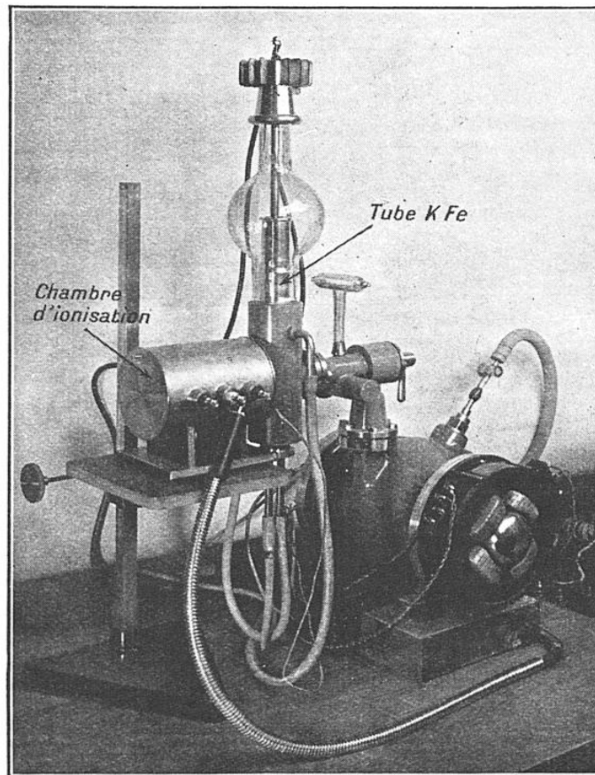
FIG. 10. — VOICI UN AUTRE TUBE A VIDE PRODUISANT LA RADIATION K DU FER (2 ANGSTRÖMS)
