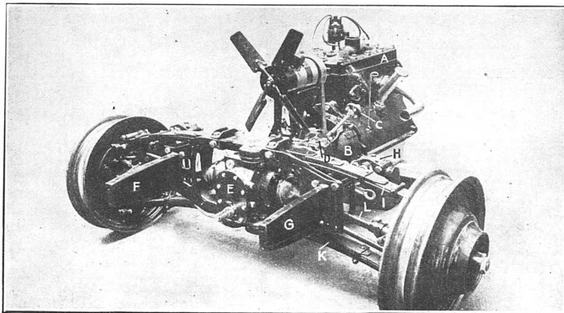
FIG. 1. — VOICI L'ENSEMBLE MOTEUR-ESSIEU-AVANT D'UNE VOITURE DE SÉRIE A ROUES AVANT MOTRICES ET A SUSPENSION PAR ROUES INDÉPENDANTES
