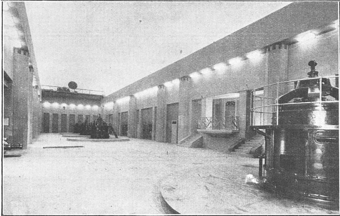
FIG. 4. — VUE INTÉRIEURE DE L'USINE, SITUÉE A 265 MÈTRES SOUS TERRE
