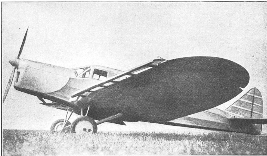
FIG. 3. — LE TRIPLACE DE TOURISME « P.-Z. 4-19 » ÉQUIPÉ D'UN MOTEUR GIPSY 100-120 CH EST UNE DES DERNIÈRES RÉALISATIONS DE L'AVIATION POLONAISE
