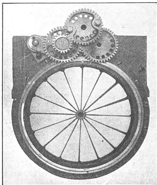
FIG. 5. — L'OBTURATEUR A LAMES RADIALES CONSTITUE LE DERNIER CRI DU PROGRÈS. Il convient pour des objectifs allant jusqu'à 12 centimètres de diamètre. Il permet le 1/150 e de seconde et son rendement lumineux est de 70 %. Les lames tournent d'abord de 90°, marquent ensuite un temps d'arrêt correspondant au temps de pose, puis reviennent en arrière de 90°.
