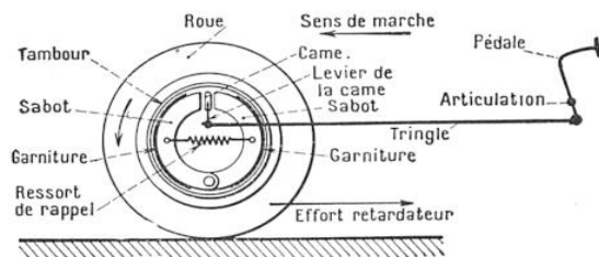
FIG. 5. — SCHÉMA DU MÉCANISME DE FREINAGE D'UNE AUTOMOBILE
