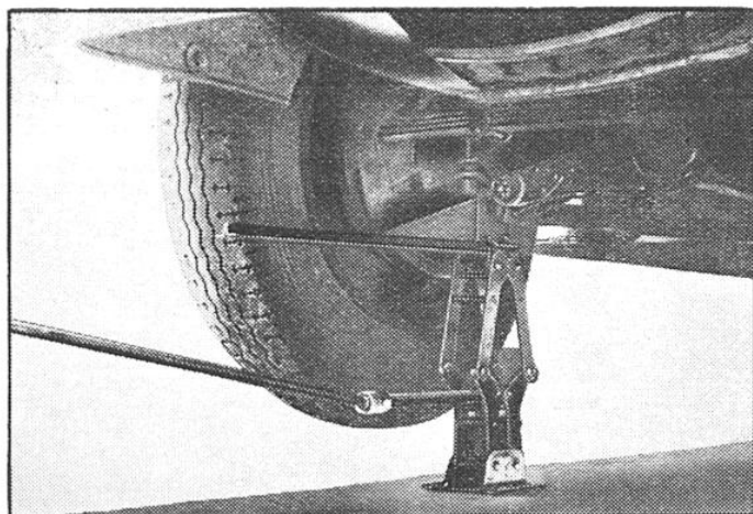
FIG. 3. — LE CRIC « SURBAISSÉ » SE GLISSE AISÉMENT SOUS LA VOITURE ET LA SOULÈVE SUFFISAMMENT POUR QU'ON PUISSE EFFECTUER LA RÉPARATION
