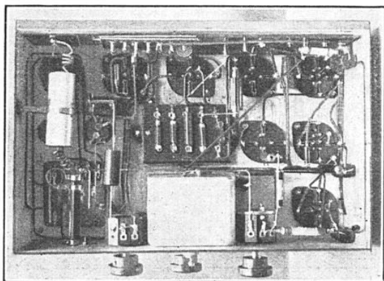
MONTAGE DU POSTE « RADIO-SOURCE »
