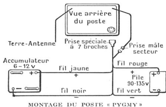
MONTAGE DU POSTE « PYGMY »
