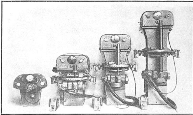
FIG. 1. — VOICI LES QUATRE MODÈLES D'APPAREILS CLASSIQUES DE PRISES DE VUES AÉRIENNES
