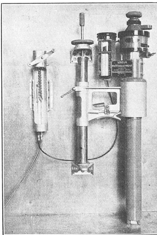
FIG. 3. — LE VISEUR, APPAREIL TOUT NOUVELLEMENT MIS AU POINT, PERMET D'ASSURER AVEC PRÉCISION ET DE FAÇON SEMI-AUTOMATIQUE, LE « POINTAGE » DE L'APPAREIL DE PRISES DE VUES
