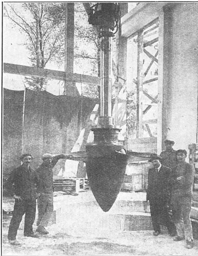
FIG. 7. — ROUES A AUBES RÉGLABLES POUR TURBINE « JEUMONT-RIVAL », ADAPTÉE A UNE CHUTE DE 4 MÈTRES ET A UN DÉBIT DE 34 MÈTRES CUBES A LA SECONDE. LE DIAMÈTRE DE CETTE ROUE EST DE 2 M 80
