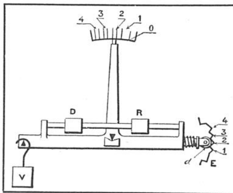
FIG. 4. — PRINCIPE DU « DÉCLENCHÉUR » QUI ACTIONNE AUTOMATIQUEMENT LE CHANGEMENT DE VITESSE
