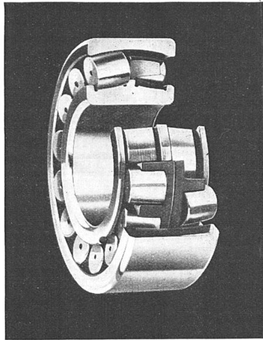
FIG. 4. — ROULEMENT A ROTULE
