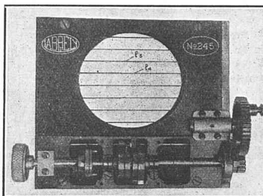
FIG. 4. — VUE DE FACE DE L'OBTURATEUR A PERSIENNE
