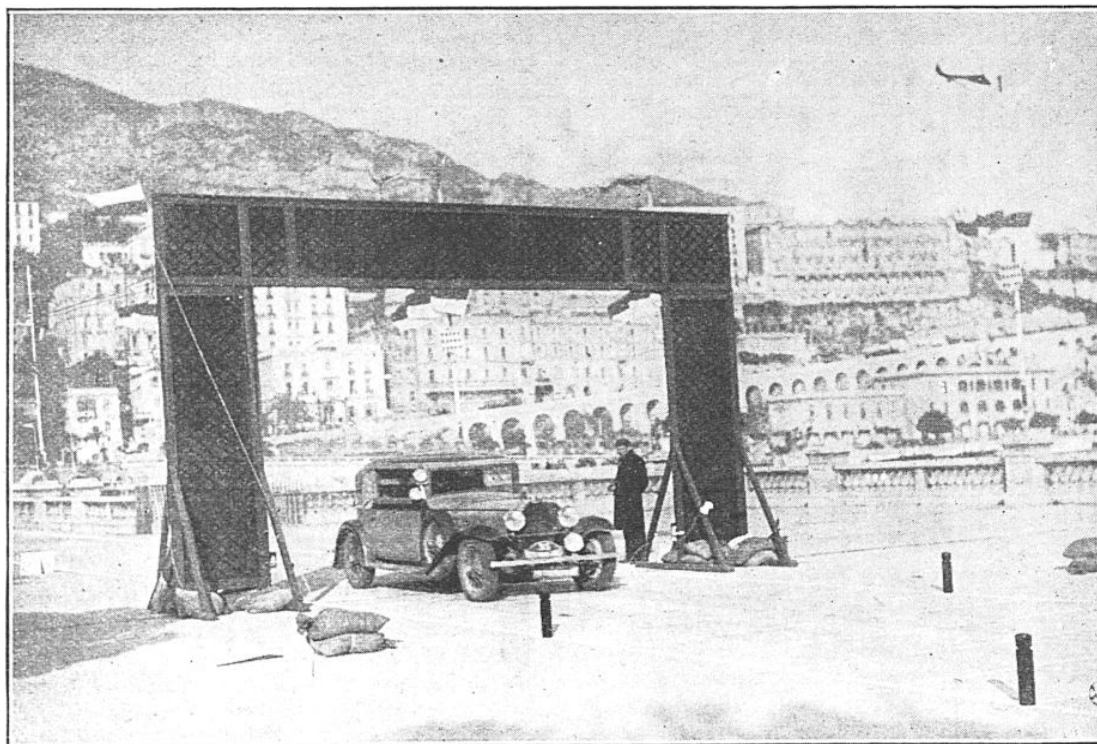
FIG. 7. — INSTALLATION DE CHRONOMÉTRAGE, D'APRÈS LE SCHÉMA PRÉCÉDENT (FIG. 6), POUR L'ÉPREUVE D'ACCÉLÉRATION ET DE FREINAGE DU RALLYE DE MONTE-CARLO
