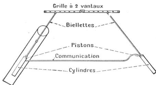
DISPOSITIF D'OUVERTURE DES PORTES
