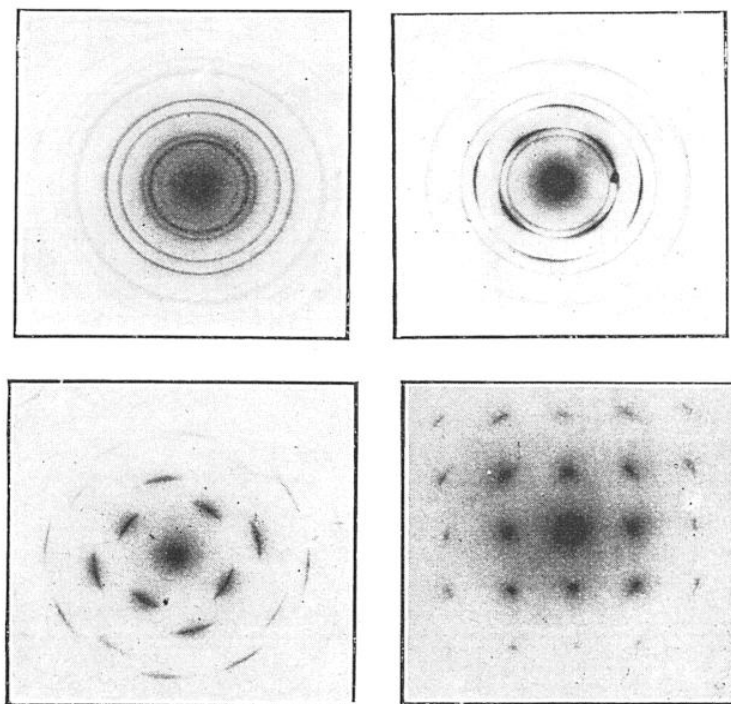
FIG. 5. — VOICI DIFFÉRENTS DIAGRAMMES ÉLECTRONIQUES (ÉLECTRONS DE 40 KILOVOLTS)
