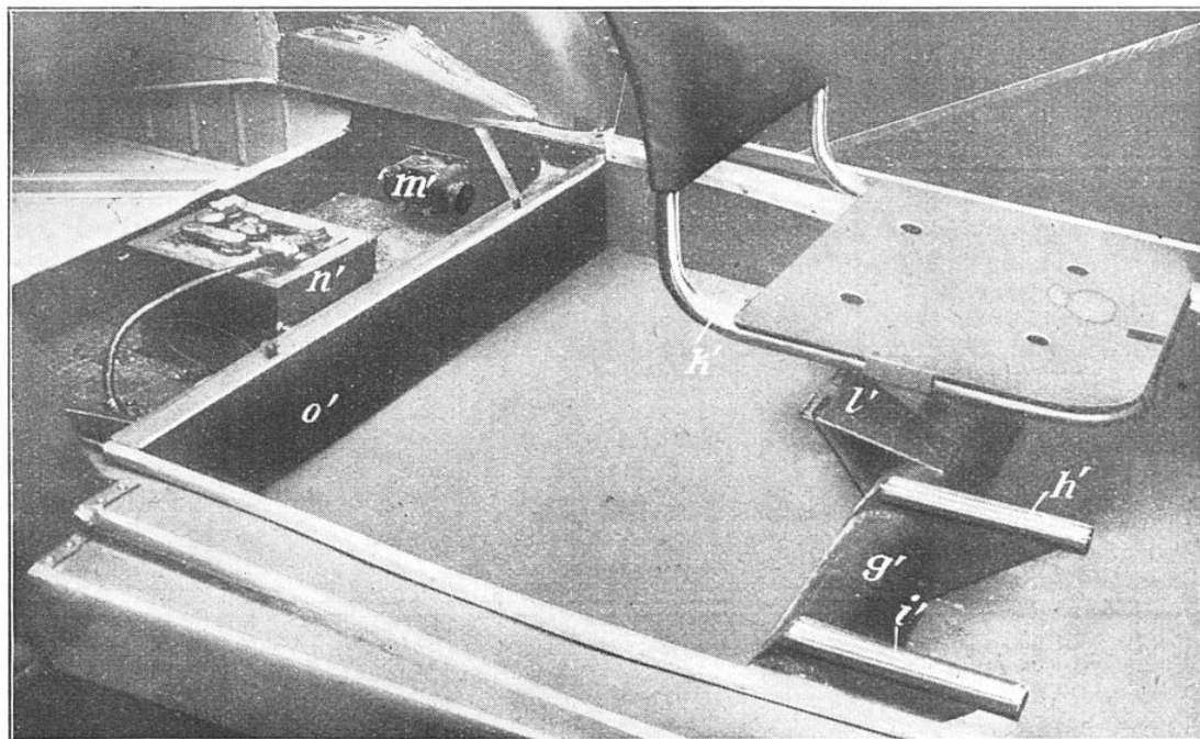
FIG. 3. — LE CHASSIS-CAISSON PERMET DE RÉALISER UNE CARROSSERIE TRÈS BASSE, QUI ASSURE UNE MEILLEURE TENUE DE ROUTE EN RÉALISANT UNE « LIGNE » PLUS MODERNE. On voit ici le montage des sièges avant. Les sièges K' sont portés sur des guides h' par le tube g', qui sert en même temps d'entretoise pour le châssis-caisson. La batterie d'accumulateurs u' est logée derrière la traverse O' du caisson. Aucun organe mécanique ne gêne les passagers, qui peuvent poser les pieds directement sur la plaque de base du châssis qui peut être très rapprochée du sol.
