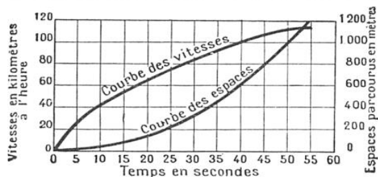
FIG. 1. — DIAGRAMME D'UN ESSAI D'ACCÉLÉRATION D'UNE VOITURE AUTOMOBILE
