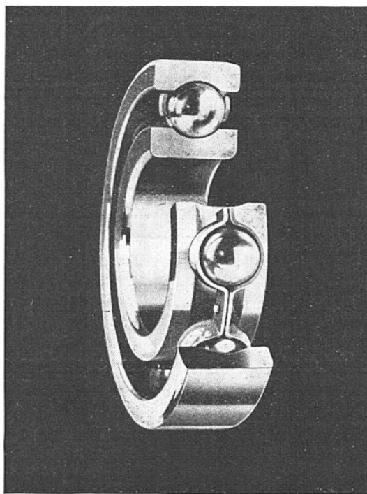
FIG. 2. — VUE D'UN ROULEMENT À BILLES OU CELLES-CI SONT MAINTENUES DANS UNE CAGE FORMÉE DE DEUX PARTIES RIVÉES. Si on laissait les billes libres dans leur chemin de roulement, en contact les unes après les autres, cela provoquerait entre elles des pressions et des frottements. C'est pourquoi on les maintient séparées les unes des autres au moyen de cages.
