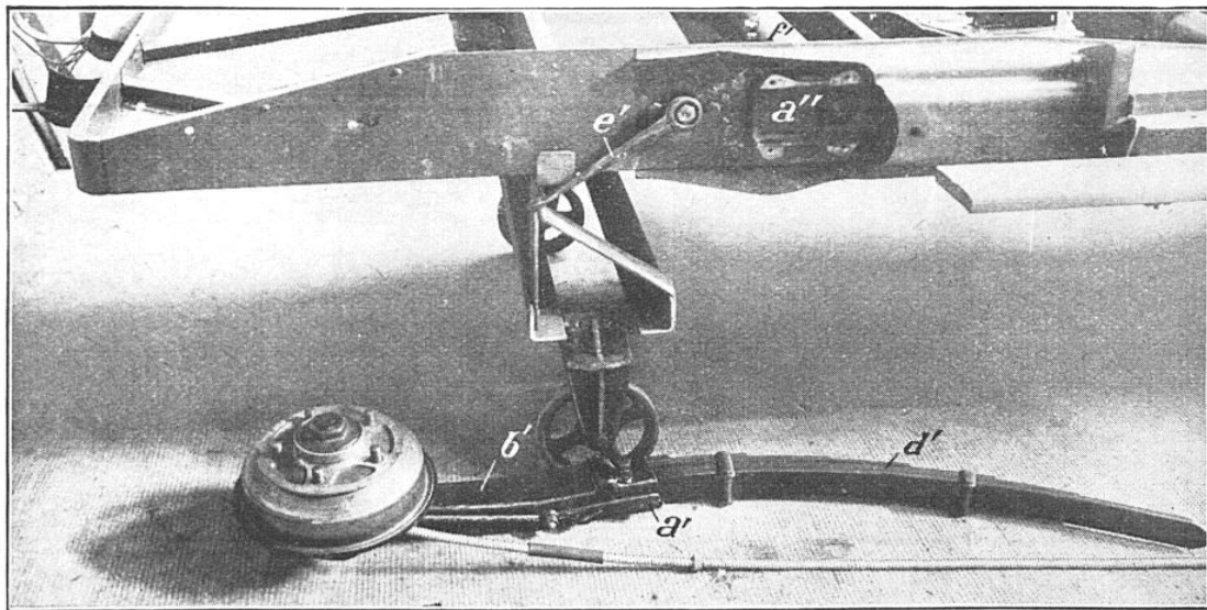
FIG. 2. — CHASSIS-CAISSON CONSTITUANT EN MÊME TEMPS LA BASE DE LA CARROSSERIE Dans les voitures ordinaires, le cadre de la carrosserie se superpose au châssis de la voiture, dont il est indépendant. Dans une voiture moderne, il est avantageux de combiner ces deux éléments en un seul, comme on le voit sur cette figure qui représente la partie arrière d'un châssis d'automobile constituant en même temps le cadre de la carrosserie : le ressort de suspension d' vient, par l'embase a', se raccorder en a'' sur ce châssis. Le levier e est le levier de commande de l'amortisseur que l'on voit à gauche.
