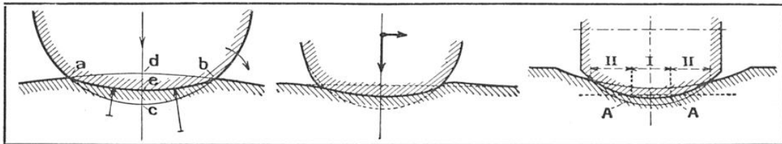
FIG. 1. — VOICI LES CAUSES PRINCIPALES DU « FROTTEMENT DE ROULEMENT »
