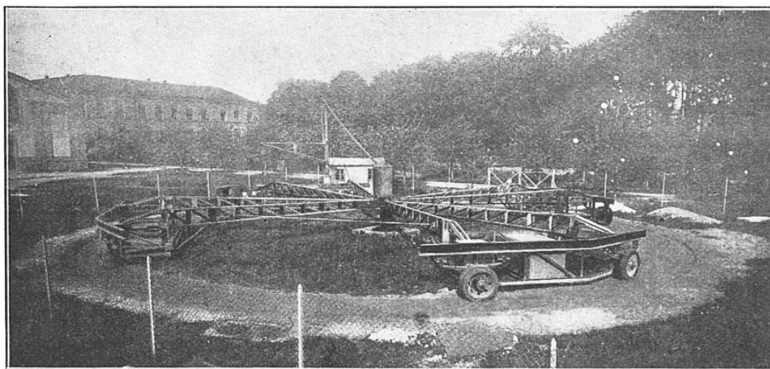
CARROUSEL DE 20 MÈTRES DE DIAMÈTRE POUR L'ÉTUDE DES REVÊTEMENTS DES ROUTES
