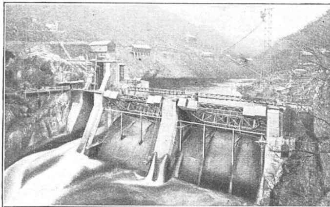
FIG. 3. — LE BARRAGE DÉVERSOIR DE LA CADÈNE
