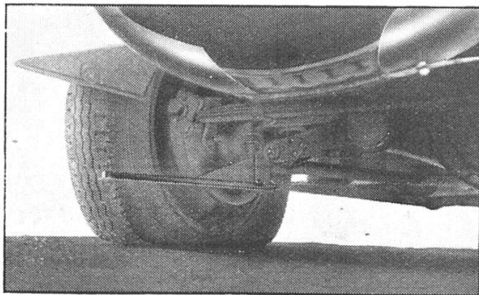
FIG. 1. — L'AFFAISSEMENT D'UN PNEU SUPERCONFORT, LORS D'UNE CREVAISON, REND EXTRÊMEMENT DIFFICILE LE PLACEMENT D'UN CRIC ORDINAIRE
