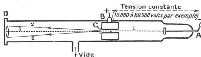
FIG. 2. — SCHÉMA D'UN APPAREIL POUR L'ANALYSE AU MOYEN DE LA DIFFRACTION DES ÉLECTRONS
