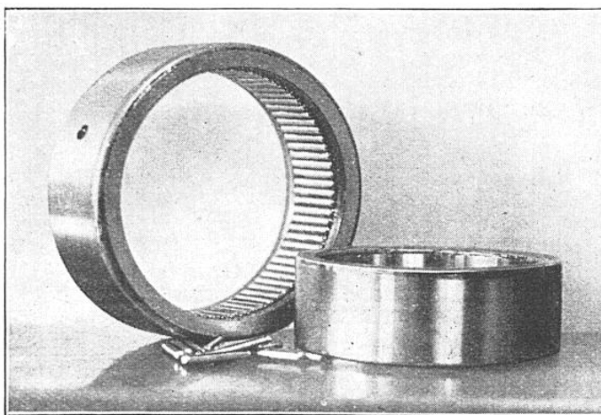
FIG. 10. — ASPECT D'UN ROULEMENT À AIGUILLES DÉMONTÉ : À DROITE, CHEMIN DE ROULEMENT INTÉRIEUR
