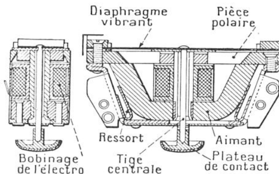
FIG. 1. — COMMENT EST CONSTITUÉ L'APPAREIL PERMETTANT AUX SOURDS D'ENTENDRE PAR CONDUCTION OSSEUSE
