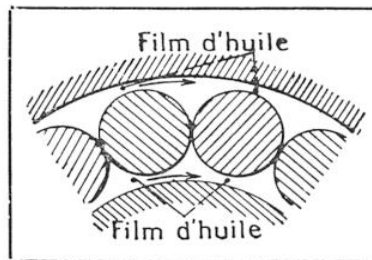
FIG. 11. - COMMENT FONCTIONNE UN ROULEMENT A AIGUILLES
