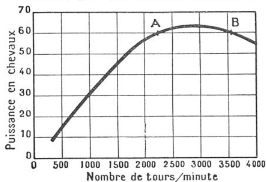
FIG. 2. — LA PUISSANCE D'UN MOTEUR EST FONCTION DE SON « NOMBRE DE TOURS » Voici une courbe-type donnant cette puissance en fonction du nombre de tours. La zone comprise entre A et B est la zone de meilleure utilisation du moteur, correspondant à la puissance maxima.
