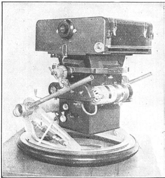
FIG. 8. — LE PLUS MODERNE ET LE PLUS PRÉCIS DES APPAREILS A PLAQUES
