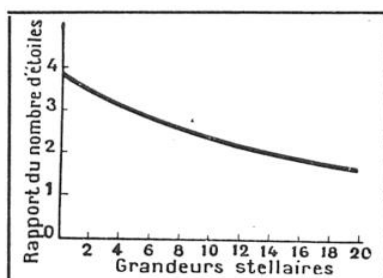
FIG. 1. — LE RAPPORT DU NOMBRE D'ÉTOILES DÉCROÎT CONSTAMMENT AVEC LES GRANDEURS STELLAIRES
