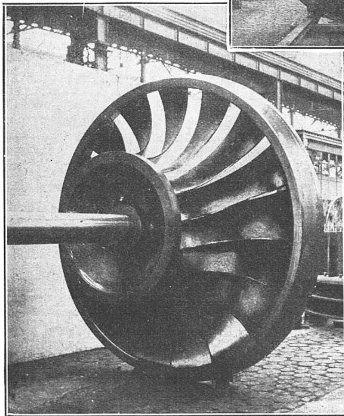
FIG. 2. — ROUE D'UNE TURBINE « FRANCIS », A AUBES ÉTROITES, TOURNANT A 400 TOURS-MINUTE
