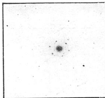
FIG. 6. — CRISTAL UNIQUE DE PARAFFINE (ÉLECTRONS DE 40 KILOVOLTS)
