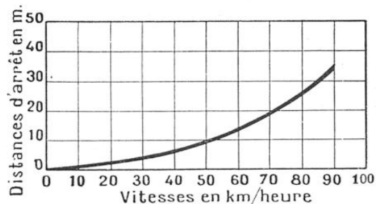
FIG. 4. — COURBE DE FREINAGE-TYPE D'UN VÉHICULE AUTOMOBILE
