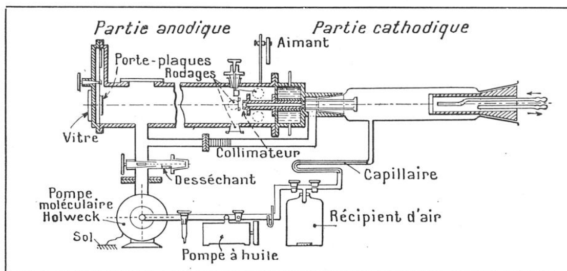
FIG. 3. — SCHÉMA D'UN APPAREIL POUR L'ÉTUDE DE LA DIFFRACTION DES ÉLECTRONS, MIS AU POINT PAR M. J.-J. TRILLAT, DANS LES LABORATOIRES DE M. MAURICE DE BROGLIE. A droite, la partie productrice d'électrons (cathode) portée à un potentiel négatif de l'ordre de 30 à 50 kilovolts. A gauche, partie anodique (chambre de diffraction) mise au sol.
