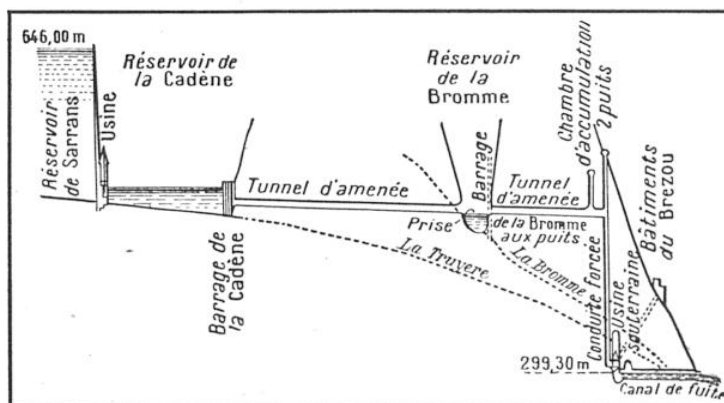
FIG. 2. — PROFIL EN LONG DE L'AMÉNAGEMENT HYDROÉLECTRIQUE DE LA TRUYÈRE ET DE LA BROMME
