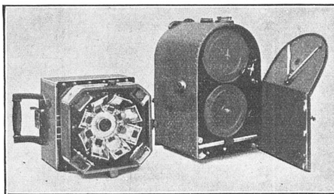
FIG. 10. — VOICI, DÉMONTÉ, L'APPAREIL PANORAMIQUE ALLEMAND QUI PERMET DE PRENDRE A TRÈS PETITE ÉCHELLE UNE ÉTENDUE DE TERRAIN DE 30 KM CARRÉS
