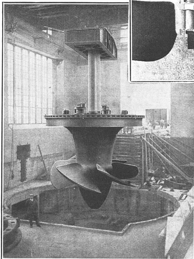
FIG. 5. — ROUE À HÉLICE DE L'UN DES GROUPES TURBO-ALTERNATEURS DE 36.600 CH DE LA CENTRALE DE KEMBS
