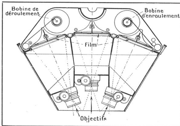
FIG. 6. — SCHÉMA D'UN APPAREIL MODERNE DE PRISES DE VUES A TROIS OBJECTIFS QUI PERMET DE PRENDRE CENT GROUPES DE TROIS VUES
