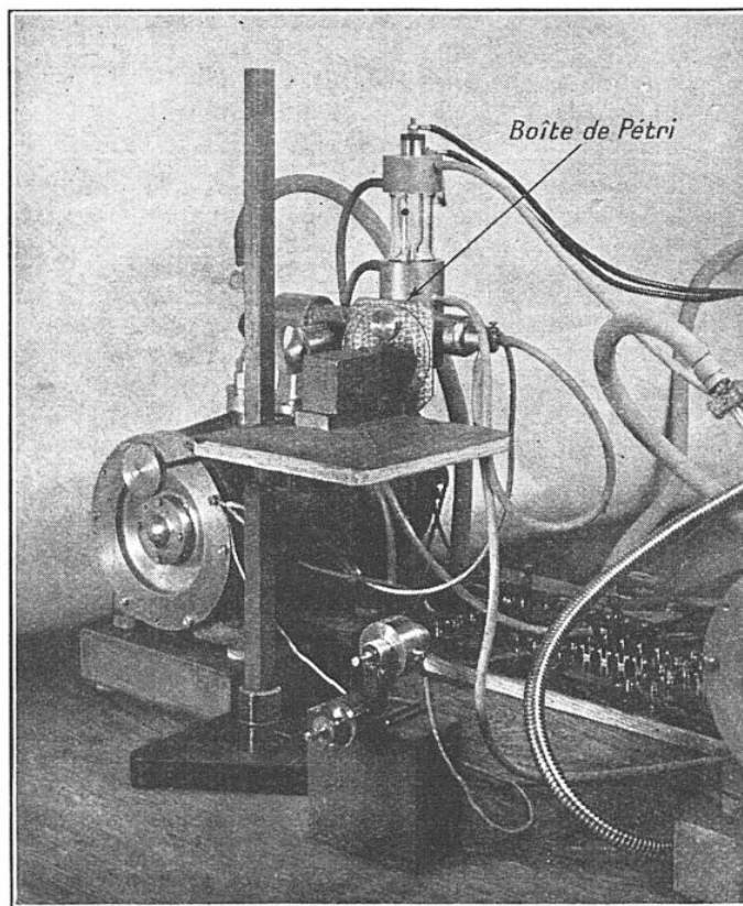
FIG. 3. — PHOTOGRAPHIE MONTRANT L'EMPLACEMENT DE LA BOÎTE DE « PÉTRI » SUR LE TUBE À RAYONS X. Les figures 9 et 10 indiquent le montage du tube lui-même.
