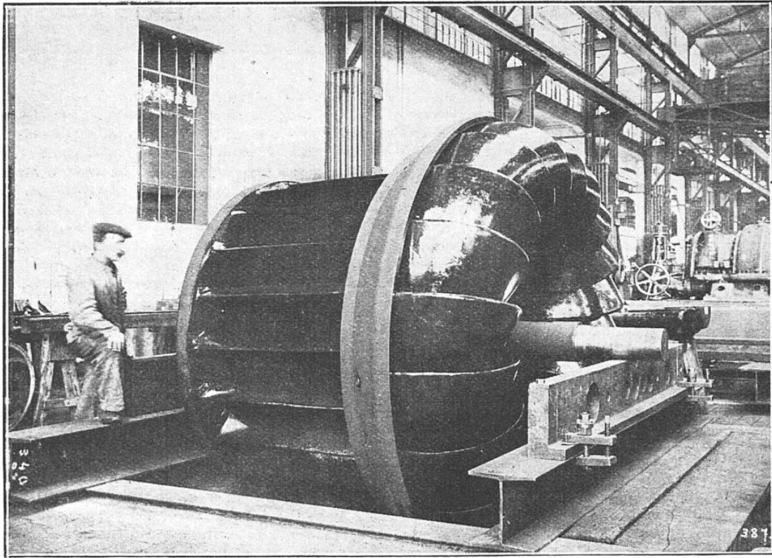
FIG. 1. — ROUE D'UNE TURBINE « FRANCIS » TOURNANT A 300 TOURS PAR MINUTE L'eau, guidée par les aubes directrices du distributeur fixe, non représenté ici, attaque la partie tournante dans le sens radial (de la périphérie vers le centre). Le mouvement de l'eau se transforme ensuite et devient axial, grâce à la forme allongée et retournée des aubes. Ce dispositif a permis d'accroître la vitesse de rotation de la turbine de façon à entraîner directement l'alternateur, à la vitesse convenable pour son rendement, sans emploi d'engrenages. Pour assurer le guidage de l'eau, il fallait, on le voit, compliquer la forme des aubes, d'où un accroissement du prix de la machine.
