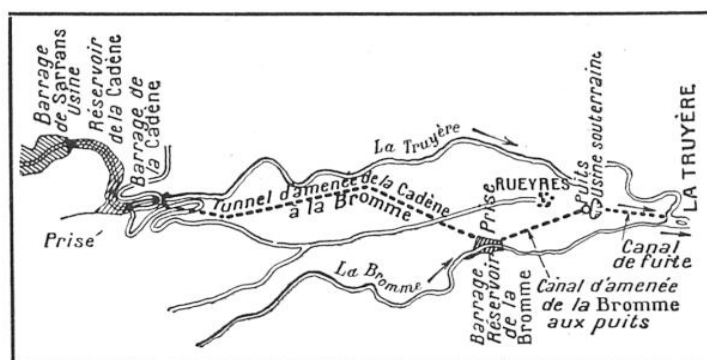
FIG. 1. — PLAN DE L'AMÉNAGEMENT HYDROÉLECTRIQUE DE LA TRUYÈRE ET DE LA BROMME
