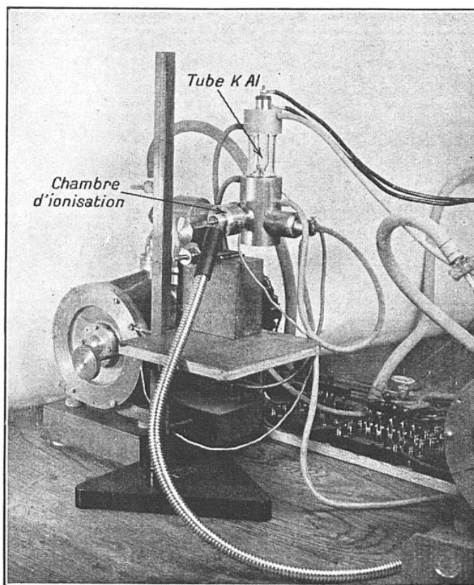
FIG. 9. — VOICI LE TUBE A VIDE QU'ON UTILISE POUR PRODUIRE LES RAYONS X DE LONGUEUR D'ONDE DE HUIT ANGSTROMS (RAIE K DE L'ALUMINIUM)
