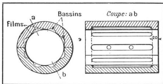
FIG. 7. — COMMENT FONCTIONNE UN DISPOSITIF A GLISSEMENT SUR COUCHE D'HUILE AU MOYEN DE BASSINS-RELAIS
