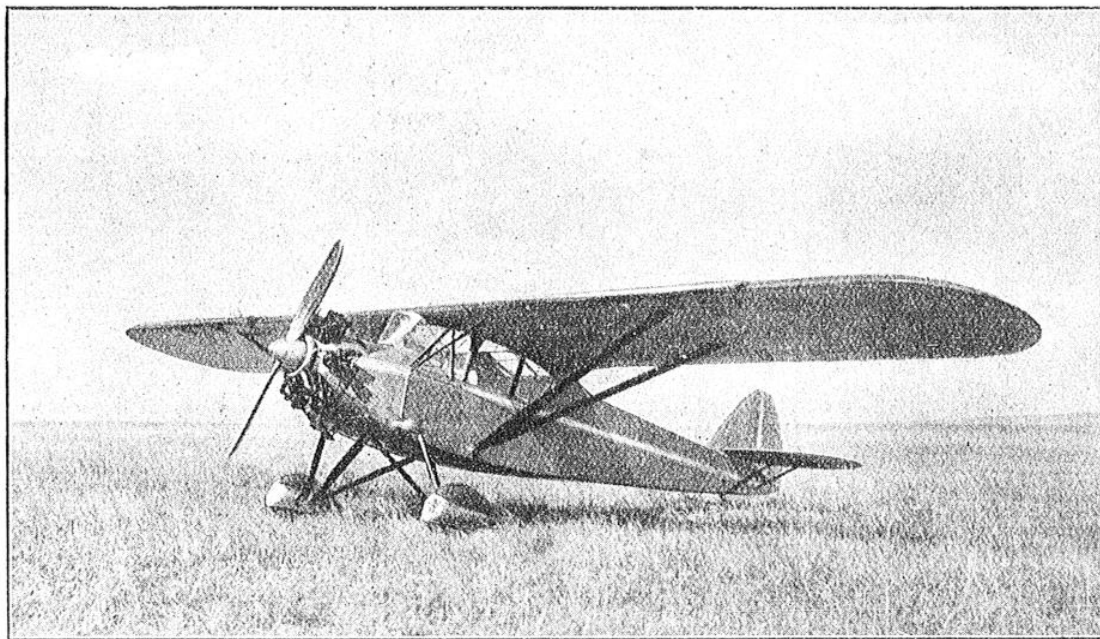
FIG. 4. — LE « POTEZ 43 », TYPE D'APPAREIL FRANÇAIS QUI RÉUNIT DES CONDITIONS DE SÉCURITÉ TOUT A FAIT INTÉRESSANTES A CELLES D'UNE TRÈS GRANDE FACILITÉ DE PILOTAGE ET QUI CONSTITUE UN DES TYPES LES PLUS ACCOMPLIS DE L'AVION DE TOURISME. La vitesse réelle de l'appareil pourrait peut-être laisser à désirer, bien qu'elle représente un gros progrès sur celle du Potez 36, frère aîné du 43. Le moteur du Potez 43 est un Potez 100 ch.
