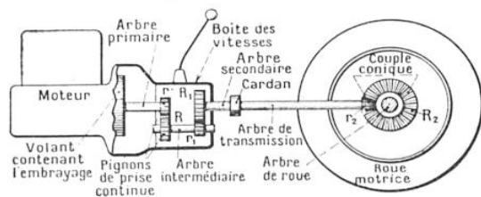
FIG. 3. — SCHÉMA DU DISPOSITIF DE DÉMULTIPLICATION PLACÉ ENTRE LE MOTEUR ET LES ROUES MOTRICES D'UNE AUTOMOBILE
