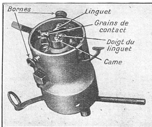
FIG. 8. — APPAREIL « DÉCLENCHÉUR » DÉROULEUR DE BANDES SERVANT AU CHRONOMÉTRAGE MÉCANIQUE
