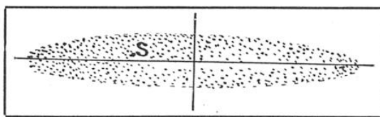
FIG. 3. — LA « GALAXIE » A LA FORME D'UN AMAS LENTICULAIRE DONT L'ÉPAISSEUR EST COMPRISE ENTRE 15.000 ET 30.000 ANNÉES DE LUMIÈRE ET DONT LA LONGUEUR MESURE ENVIRON 150.000 ANNÉES DE LUMIÈRE
