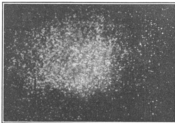
FIG. 2. — L'AMAS GLOBULAIRE DU CENTAURE, LE PLUS RAPPROCHÉ DE NOUS, EST CEPENDANT SITUÉ À UNE DISTANCE DE 20.000 ANNÉES DE LUMIÈRE
