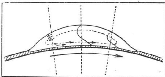
FIG. 8. — LE GLISSEMENT SUR FILM D'HUILE, A BASSINS-RELAIS, EST UN VÉRITABLE ROULEMENT SUR HUILE
