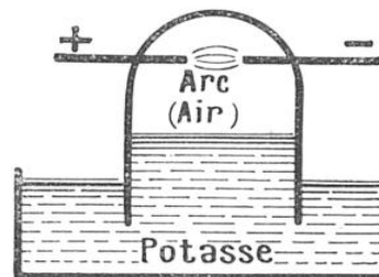
FIG. 6. — L'EXPERIENCE PAR LAQUELLE CAVENDISH ANALYSA L'AIR, AVANT LAVOISIER
