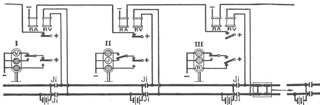
FIG. 3. — SCHÉMA DU BLOCK AUTOMATIQUE LUMINEUX
