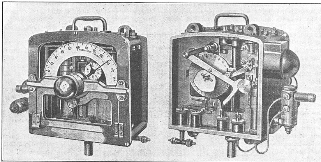
FIG. 5. — LES APPAREILS « FLAMAN » ET « RODOLAUSSE » RÉUNIS
