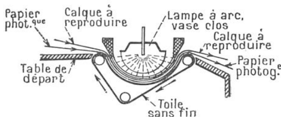
FIG. 1. — SCHÉMA D'UN CHÂSSIS À DÉROULEMENT CONTINU POUR LA REPRODUCTION AUTOMATIQUE DES PLANS
