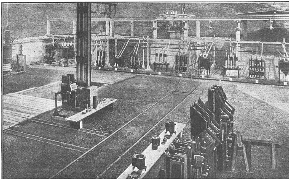
FIG. 7. — LE PROBLÈME DE LA COUPURE DE PUISSANCES ÉLEVÉES PRÉSENTE UNE TELLE IMPORTANCE DANS LA PRODUCTION DE L'ÉNERGIE ÉLECTRIQUE QUE LES SERVICES D'ESSAIS DES DISJONCTEURS NÉCESSITENT UN MATÉRIEL CONSIDÉRABLE
