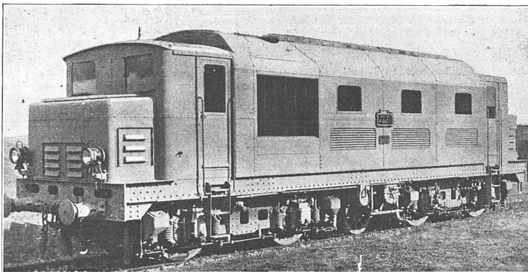
FIG. 5. — TYPE DE LOCOMOTIVE A MOTEUR DIESEL ET TRANSMISSION ÉLECTRIQUE, UTILISÉE POUR MANŒUVRES PAR LES CHEMINS DE FER DE CEINTURE
