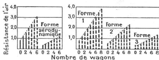
FIG. 4. — SCHÉMA DONNANT LA VALEUR DE LA RÉSISTANCE DE L'AIR EN FONCTION DU NOMBRE DE WAGONS, POUR LES TRAINS DONT LES FORMES ONT ÉTÉ DONNÉES SUR LA FIGURE PRÉCÉDENTE
