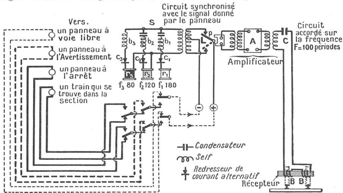
FIG. 9. — L'INSTALLATION DU « CAB SIGNAL » A BORD DE LA LOCOMOTIVE
