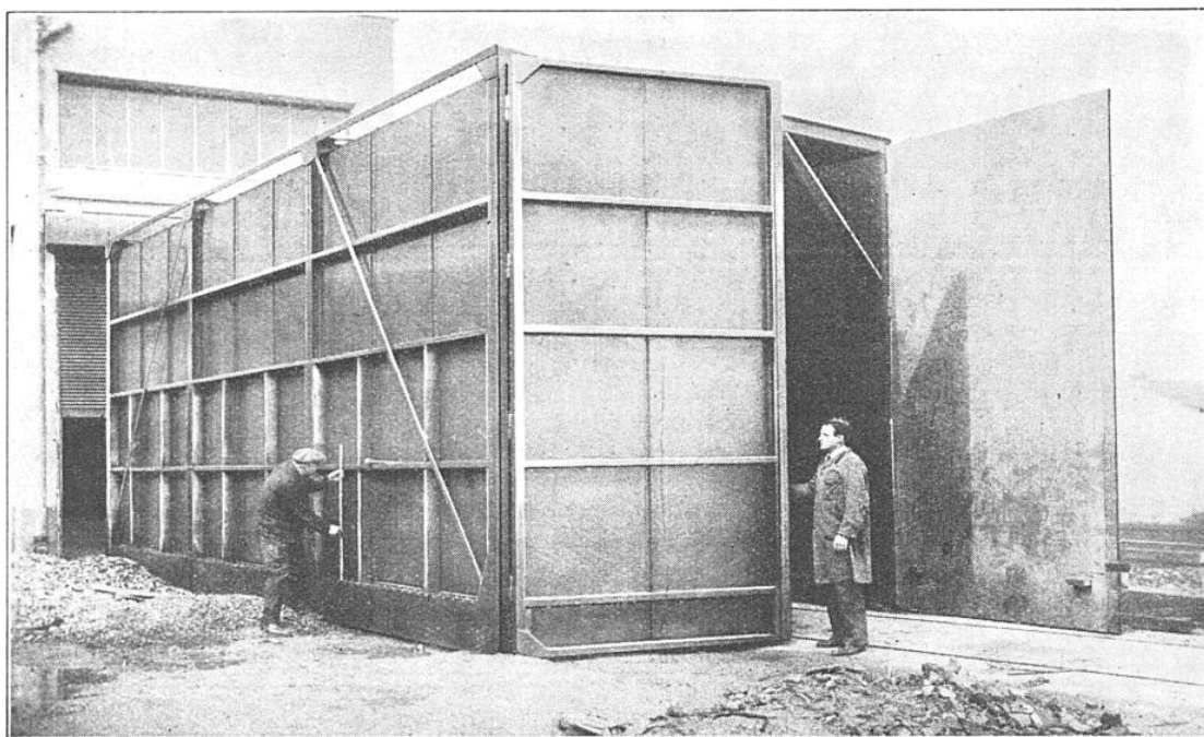
FIG. 7. — VOICI UNE CHAMBRE D'ESSAIS POUR WAGONS FRIGORIFIQUES, EN COURS D'INSTALLATION, AU LABORATOIRE CRYOGÈNE DE L'OFFICE NATIONAL DES RECHERCHES SCIENTIFIQUES ET INDUSTRIELLES ET DES INVENTIONS, A BELLEVUE (SEINE-ET-OISE)
