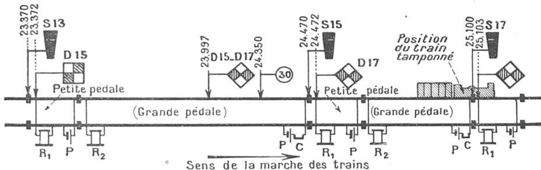
FIG. 4. — BLOCK AUTOMATIQUE A SIGNAUX MÉCANIQUES (CAS DU RÉSEAU DE L'EST)
