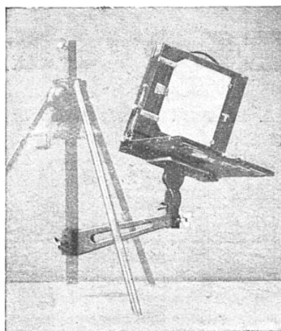
Dispositif pour photographier au ras du sol
