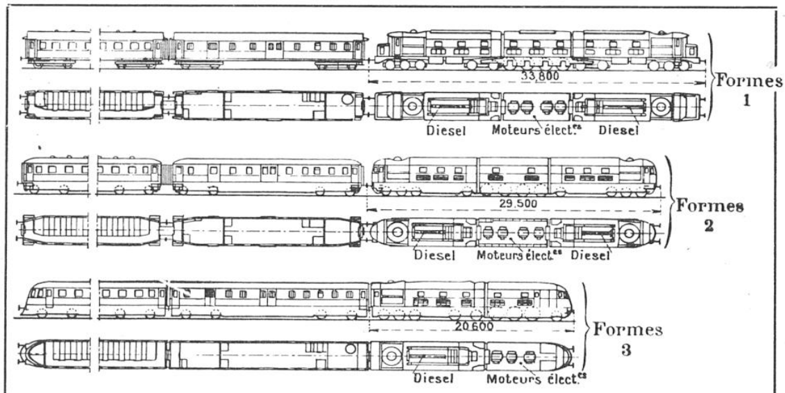
FIG. 3. — RÉSULTATS DES EXPÉRIENCES FAITES, AUX ÉTATS-UNIS, SUR LA RÉSISTANCE QUE L'AIR OPPOSE À LA MARCHÉ DE TOUT UN TRAIN À LOCOMOTIVE DIESEL ÉLECTRIQUE
