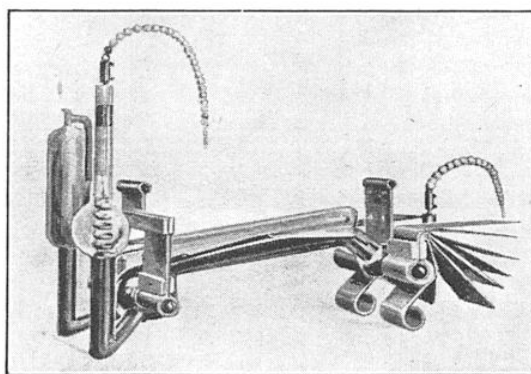
FIG. 3. — LAMPE A VAPEUR DE MERCURE EN SILICE, TYPE « HENRI GEORGE »
