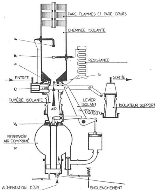
FIG. 5. — PRINCIPE DU DISJONCTEUR A AIR COMPRIMÉ DES « A. C. E. D. »
