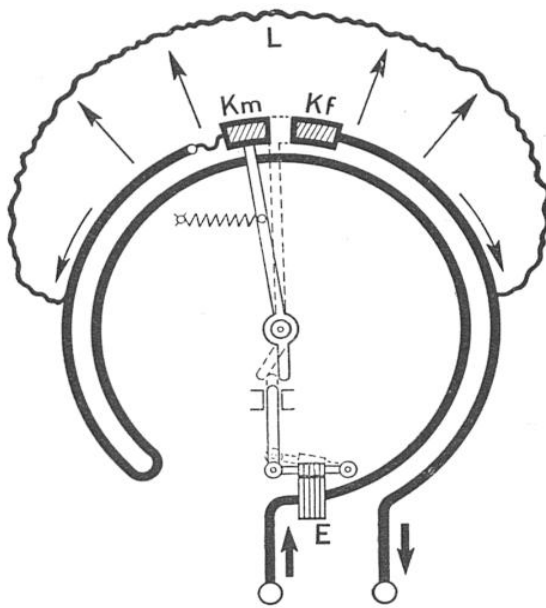
FIG. 1. — PRINCIPE DE FONCTIONNEMENT D'UN DISJONCTEUR ULTRA-RAPIDE POUR COURANT CONTINU
