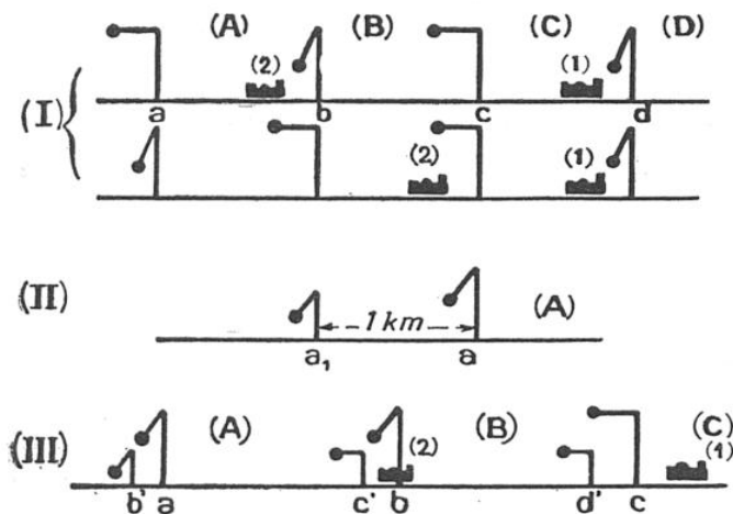
FIG. 1. — SCHÉMA DU « BLOCK-SYSTEM »
