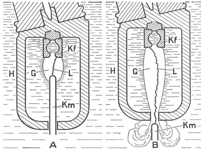
FIG. 3. — PRINCIPE DE LA CHAMBRE D'EXTINCTION DE L'ARC
