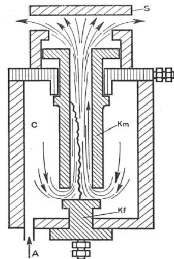
FIG. 6. — PRINCIPE DU DISJONCTEUR A AIR COMPRIMÉ A CONTACT CYLINDRIQUE
