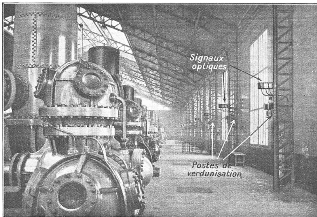
FIG. 7. — VUE D'ENSEMBLE DES POMPES DE L'USINE DE VITRY (VILLE DE PARIS)
