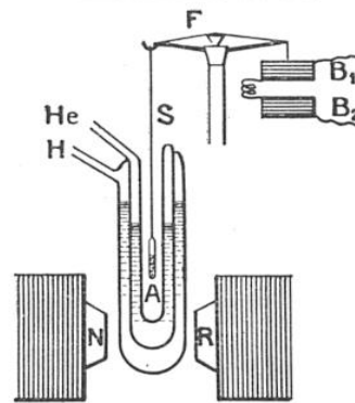
FIG. 6. — SCHÉMA DE L'EXPÉRIENCE DE M. DE HAAS, QUI A PERMIS DE RÉALISER LES TEMPÉRATURES LES PLUS BASSES JUSQU'À PRÉSENT ATTEINTES
