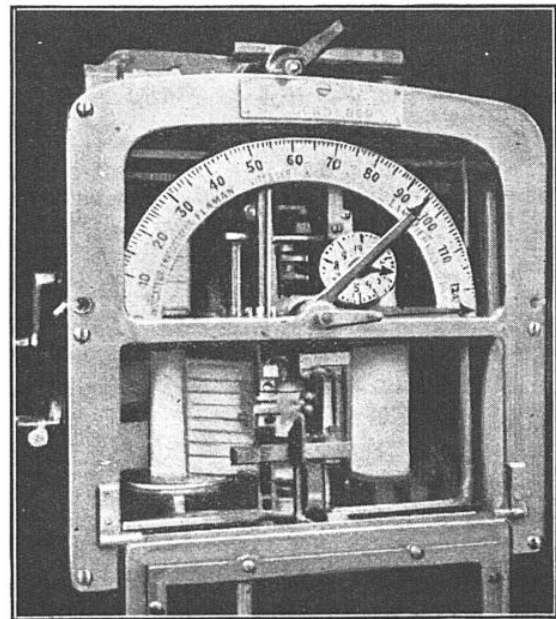
FIG. 2. — VOICI L'APPAREIL « FLAMAN », QUI EST A LA FOIS INDICATEUR DE VITESSE ET ENREGISTREUR DE SIGNAUX ACOUSTIQUES
