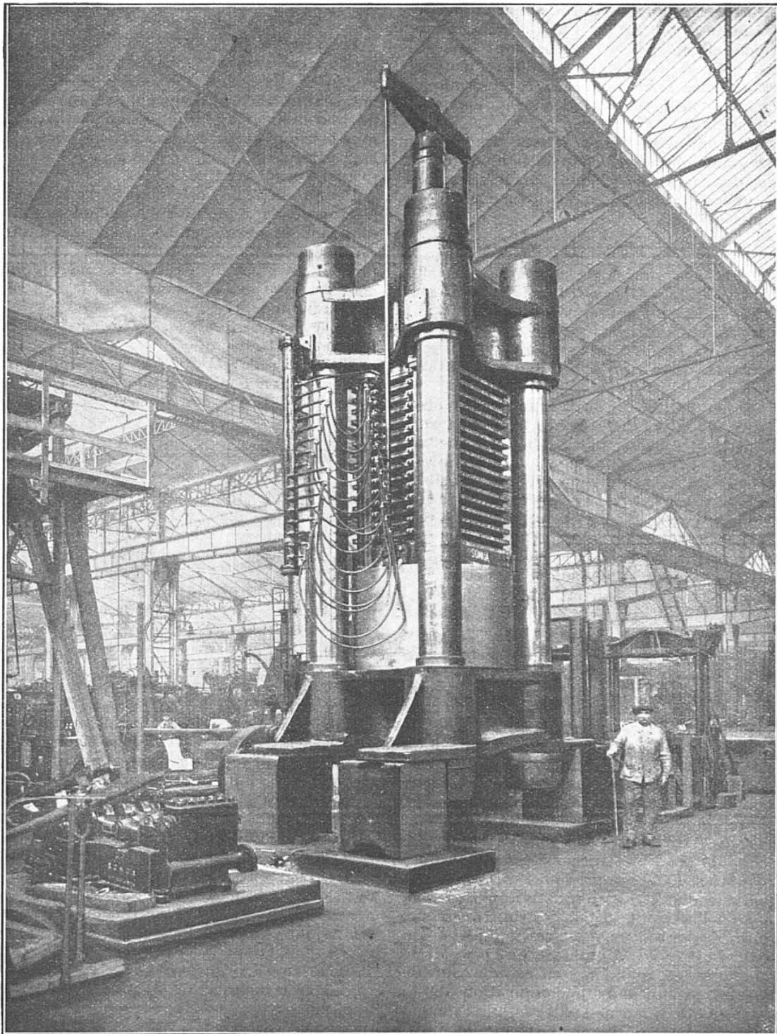
FIG. 1. - VOICI L'UNE DES PRESSES A MATIÈRES PLASTIQUES LES PLUS PUISSANTES DU MONDE Cette presse hydraulique, de construction française, a une force de 6.500 tonnes. Elle est utilisée pour le moulage des matières plastiques en plaques.
