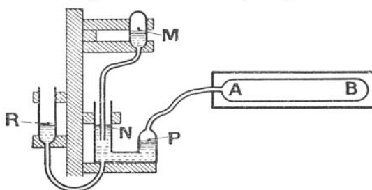
FIG. 2. — SCHÉMA DE PRINCIPE D'UN THERMOMÈTRE À GAZ « RÉEL »
