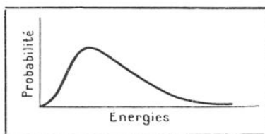
FIG. 1. — DISTRIBUTION DES ÉNERGIES DES MOLECULES D'UN GAZ PARFAIT
