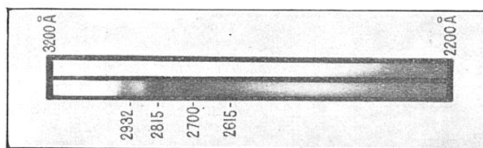
FIG. 2. — SPECTRE D'ABSORPTION DE L'ERGOSTÉROL
