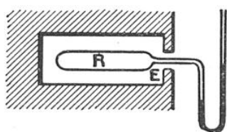
FIG. 1. — SCHÉMA DE PRINCIPE D'UN THERMOMÈTRE À GAZ
