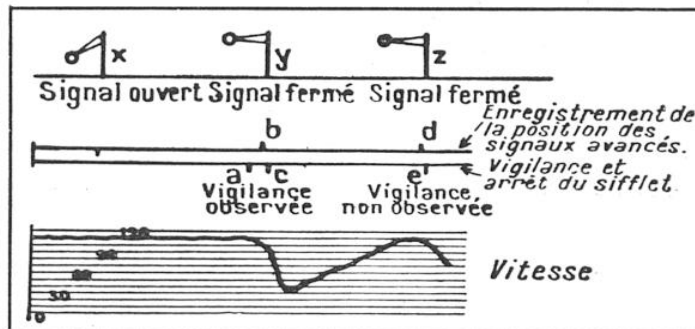
FIG. 7. — COMMENT SE PRÉSENTE L'ENREGISTREMENT DE LA POSITION DES SIGNAUX SUR UNE BANDE DE L'APPAREIL « FLAMAN » RÉGLEMENTAIRE
