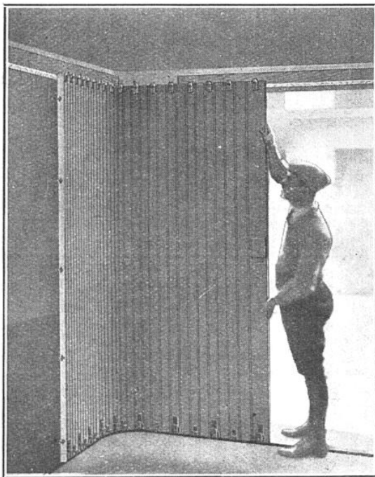
LA PORTE SOUPLE « SYSTÈME POYER »
