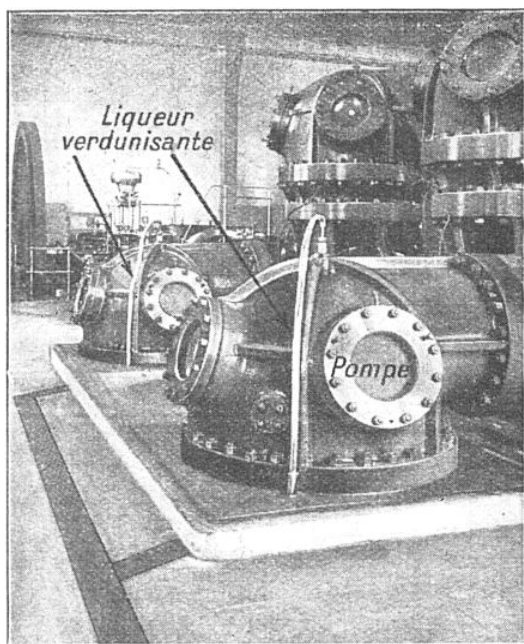
FIG. 3. — L'ARRIVÉE DE LA LIQUEUR VERDUNISANTE AU CORPS DE POMPE
