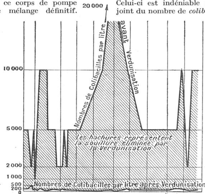
FIG. 5. — CE GRAPHIQUE MONTRE, HEURE PAR HEURE, LES NOMBRES RELATIFS DE COLIBACILLES PRÉSENTS DANS L'EAU AVANT LA VERDUNISATION (COURBE SUPÉRIEURE) ET APRÈS VERDUNISATION (COURBE INFÉRIEURE)
