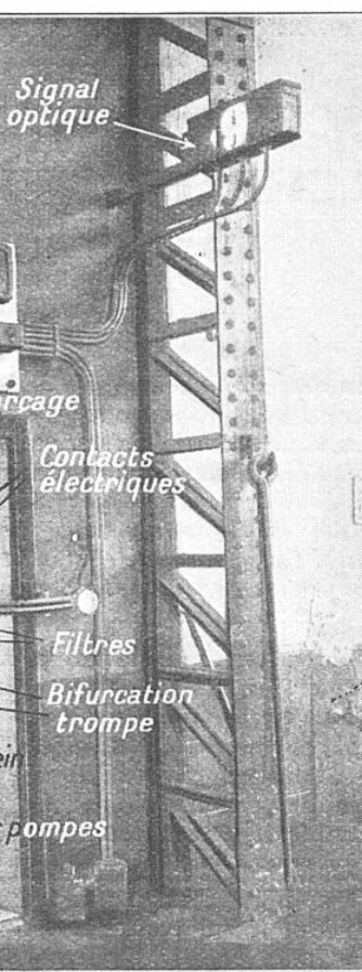
FIG. 1. — UN POSTE DE VERDUNISATION DES EAUX A L'USINE DE POMPAGE D'IVRY
