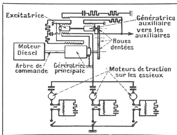
FIG. 2. — SCHÉMA DE LA DISTRIBUTION ÉLECTRIQUE DE LA LOCOMOTIVE DIESEL P.-L.-M., 920 CH
