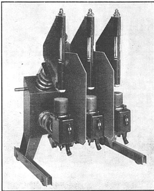
FIG. 4. — DISJONCTEUR TRIPOLAIRE DANS L'EAU POUR 24.000 VOLTS (POUVOIR DE COUPURE : 250.000 KILOVOLTS-AMPÈRES) On voit, au-dessus de la chambre de détente, l'intervalle dans l'air qui constitue le diélectrique dans la position ouverte des contacts. Les contacts mobiles sont remontés dans leurs gaines, qui en contiennent le dispositif de commande.
