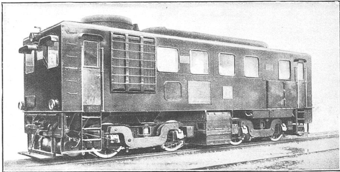
FIG. 1. — LOCOMOTIVE DIESEL ÉLECTRIQUE, DE CONSTRUCTION ALLEMANDE, DESTINÉE AU CHEMIN DE FER « SUD-MANDCHOURIEN »
