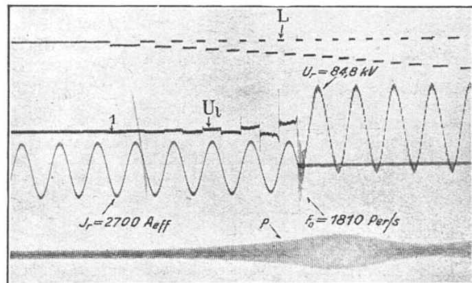
FIG. 2. — OSCILLOGRAMME DE LA COUPURE D'UN COURT-CIRCUIT AU MOYEN D'UN DISJONCTEUR DANS L'HUILE
