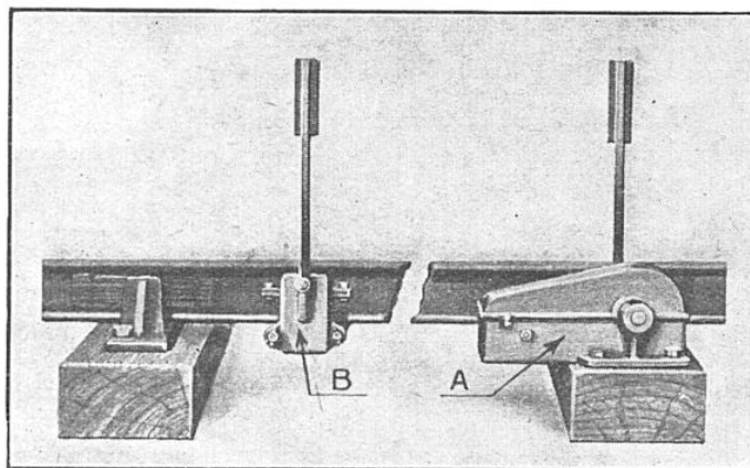
FIG. 6. — DÉCLENCHERS DE VOIE FIXÉS AUX RAILS, DANS LE SYSTÈME « RODOLAUSSE »
