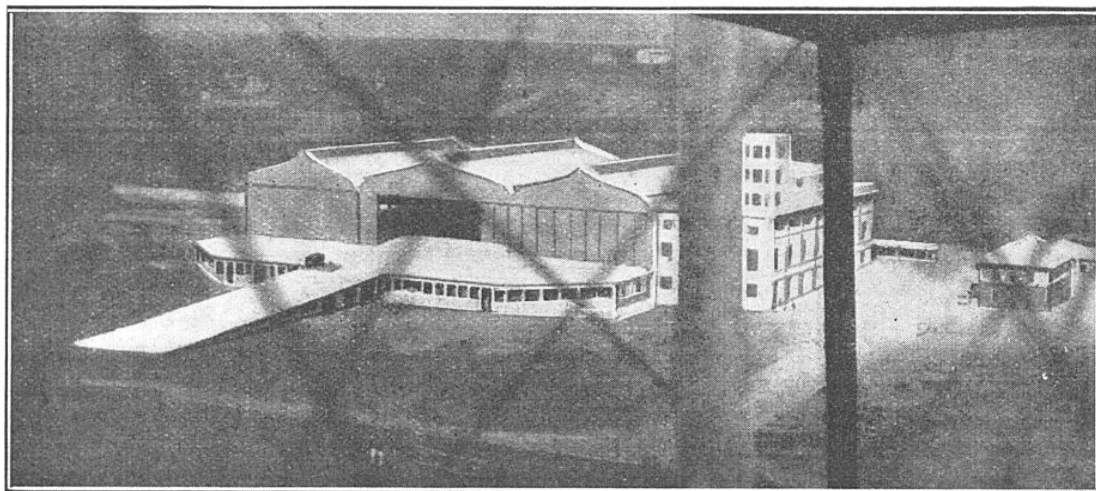
FIG. 3.- L'AÉROPORT DE LITTORIO-ROME EST ÉTABLI SUIVANT UN MODÈLE UNIQUE AU MONDE. Cet aéroport est surtout curieux du fait que son hangar est à deux étages. Le grand plan incliné qu'on voit sur ce document permet d'accéder au deuxième étage. Ce système est absolument inédit.
