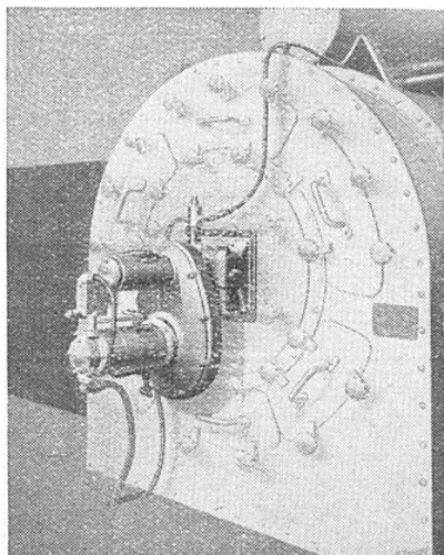
BRULEUR B 2 sur chaudière Vernon des Etabliss ts H. BOUTILLON équipé avec un MONOCOUPLEX
