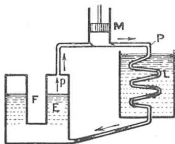
FIG. 3. — SCHÉMA D'UN « CYCLE » DE LIQUÉFACTION
