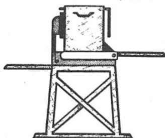
MACHINE à faire les agglomérés. 464 francs . — Faites vous-mêmes les agglomérés des parois et des cloisons de vos constructions métalliques. (Notice 197)
