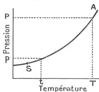
FIG. 5. — COURBE DES TENSIONS DE VAPEURS SATURANTES
