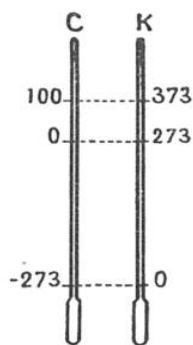
FIG. 4. — SCHÉMA MONTRANT LA CORRESPONDANCE DES ÉCHELLES CENTÉSIMALE (C) ET KELVIN (K)
