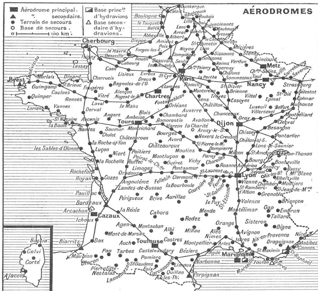
FIG. 6. — CARTE MONTRANT LA TOTALITÉ DES GRANDS AÉROPORTS ET AÉRODROMES FRANÇAIS (POUR AVIONS ET HYDRAVIONS) ET LA PRESQUE TOTALITÉ DES AÉRODROMES DE SECOURS
