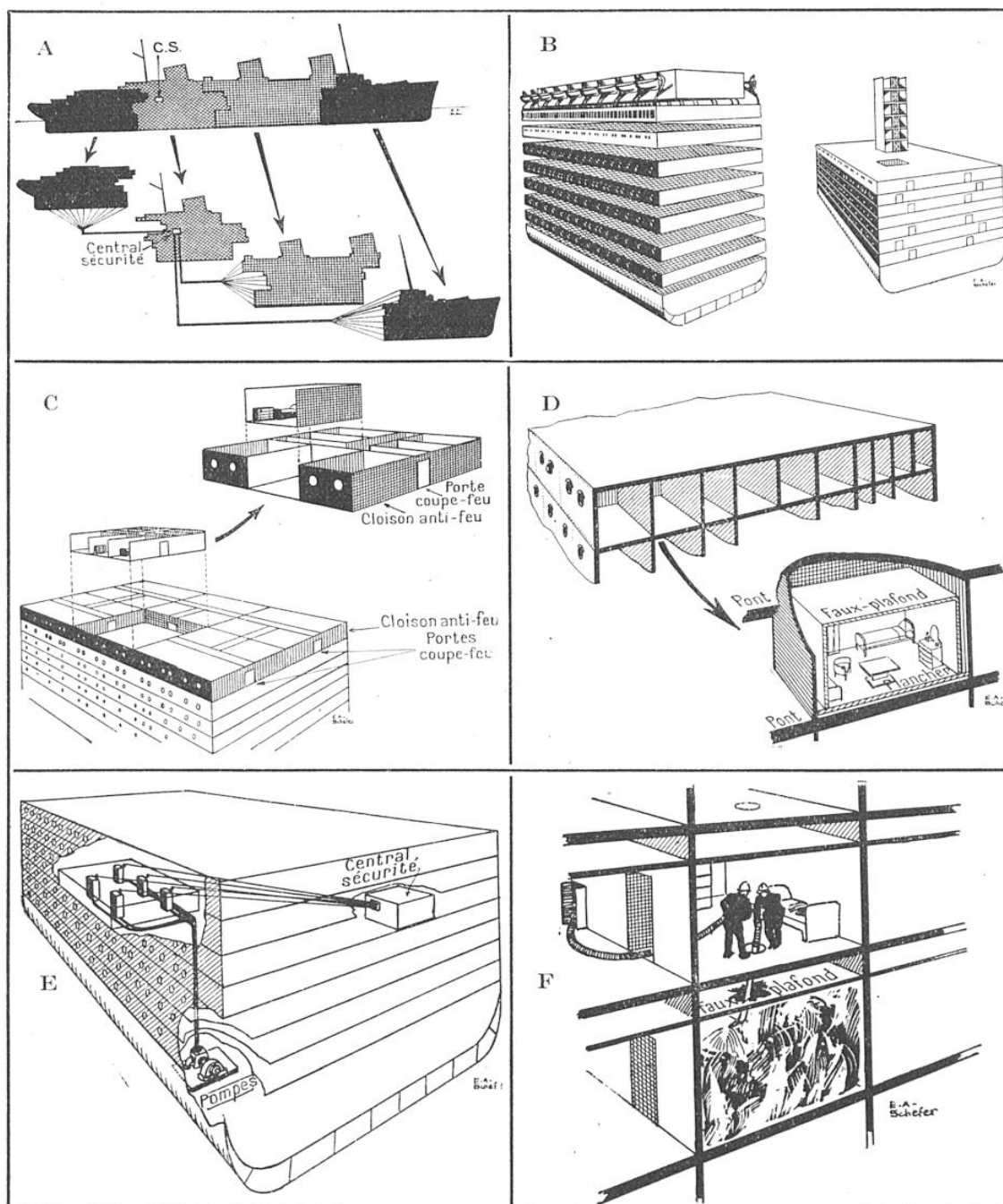
FIG. 1. — CONTRE LE FEU, LE COMPARTIMENTAGE DU PAQUEBOT « NORMANDIE » A ÉTÉ ÉTUDIÉ MINUTIEUSEMENT, COMME POUR LA PROTECTION CONTRE L'ENVAHISSEMENT PAR L'EAU
