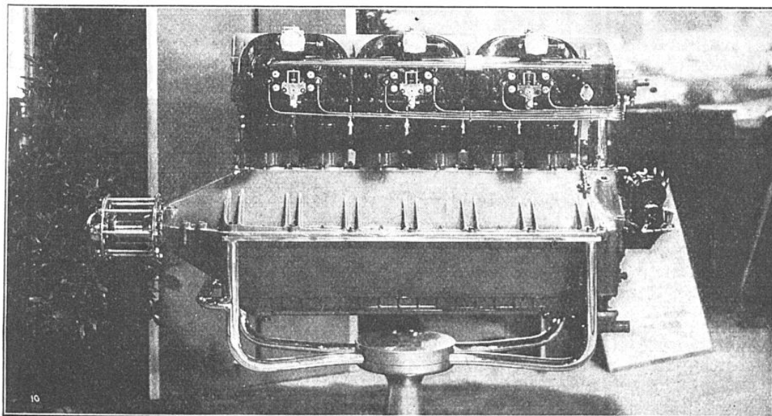
FIG. 7. — UN MOTEUR ITALIEN D'AVIATION ÉQUIPÉ DE LA CULASSE « BAGNULO », QUI LE REND APTÉ A CONSOMMER L'HUILE LOURDE. TOUT EN ASSURANT UN EXCELLENT RENDEMENT L'HUILE LOURDE PERMET D'ACCROITRE LA SÉCURITÉ, NOTAMMENT CONTRE LE FEU
