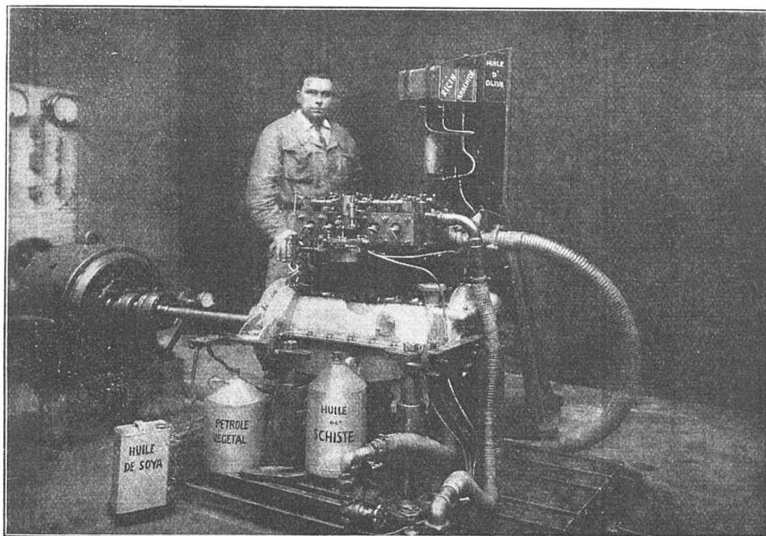
FIG. 6. — LE MOTEUR POLYCARBURANT VU DU COTÉ DE LA CULASSE SPÉCIALE « BAGNULO » (LE RESTE DU MOTEUR N'AYANT RIEN DE PARTICULIER). CETTE CULASSE PERMET D'UTILISER : LE GAZ DE GAZOGÈNE, LES ESSENCES VOLATILES ET LE GAS OIL DES HUILES VÉGÉTALES
