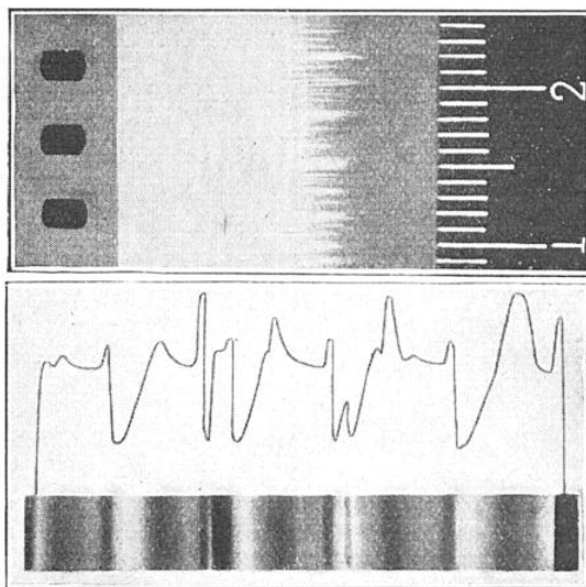
FIG. 3 ET 4. — ENREGISTREMENT SUR FILM SELON LES PROCÉDÉS A INTENSITÉ CONSTANTE OU A INTENSITÉ VARIABLE
