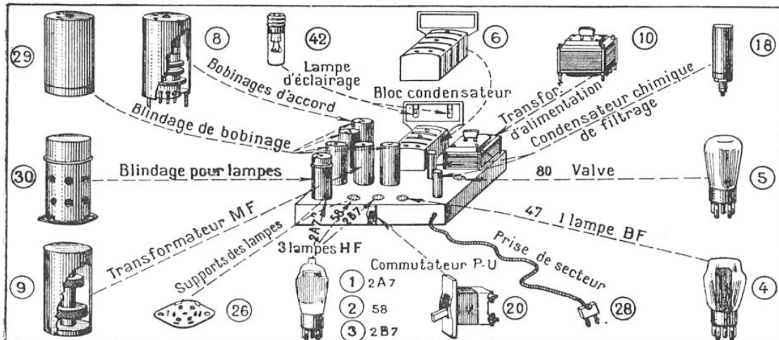
FIG. 3. — LE CHASSIS ET PIÈCES DÉTACHÉES DU POSTE QUATRE LAMPES PLUS UNE VALVE
