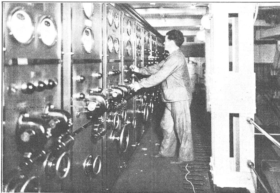
FIG. 2. — LE TABLEAU DE DISTRIBUTION D'ÉNERGIE ÉLECTRIQUE A BORD DU PAQUEBOT « NORMANDIE » PERMET, DÈS L'ALARME DONNÉE, D'ISOLER ÉLECTRIQUEMENT LA TRANCHE OU S'EST PRODUITE L'ALERTE (VOIR LE COMPARTIMENTAGE, FIG. 1)
