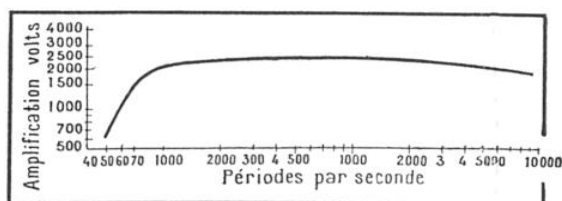
FIG. 6. — COURBE CARACTÉRISTIQUE DE L'AMPLIFICATEUR MONTRANT SA RÉPONSE LINÉAIRE ENTRE 80 ET 10.000 PÉRIODES, C'EST-A-DIRE SA FIDÉLITÉ
