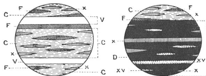
FIG. 1. — DISTRIBUTION DES TISSUS LIGNIFIÉS : A GAUCHE, DANS LA HOUILLE BRILLANTE (CLARAIN, VITRAIN) ; A DROITE, DANS LA HOUILLE MATE (DURAIN)
