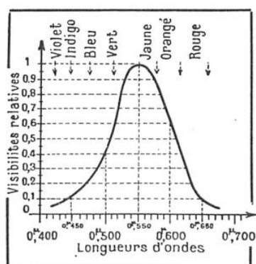
FIG. 1. — COURBE DES COEFFICIENTS DE VISIBILITÉ DES DIFFÉRENTES RADIATIONS
