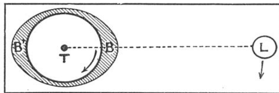
FIG. 2. — LES MARÉES EXERCENT UNE ACTION DE FREINAGE SUR LA ROTATION DE LA TERRE
