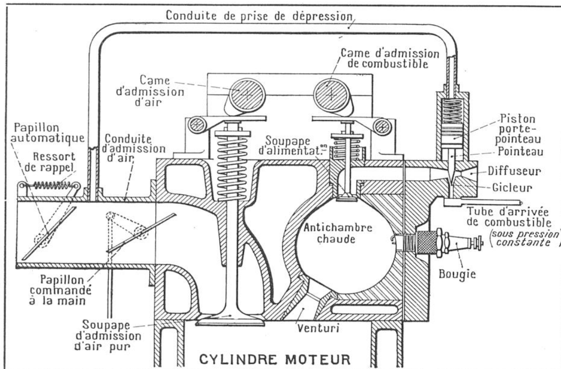
FIG. 5. — LA CULASSE DU MOTEUR POLYCARBURANT « BAGNULO »
