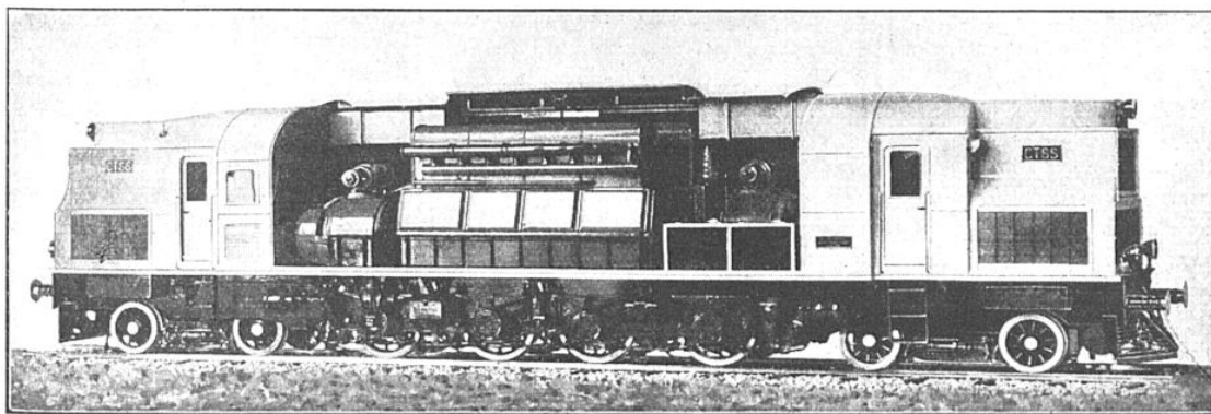
FIG. 1. - LOCOMOTIVE DIESEL ÉLECTRIQUE PROJETÉE POUR LE CHEMIN DE FER TRANSSAHARIEN D'une vitesse maximum de 90 kilomètres à l'heure, cette locomotive, qui pèse 135 tonnes, comporte deux boggies chargés à 15.250 tonnes par essieu et quatre essieux moteurs chargés chacun à 19 tonnes. Elle peut remorquer un train de marchandises de 1.500 tonnes à 45 kilomètres à l'heure, ou un train express de quatorze wagons-lits à 80 kilomètres à l'heure.
