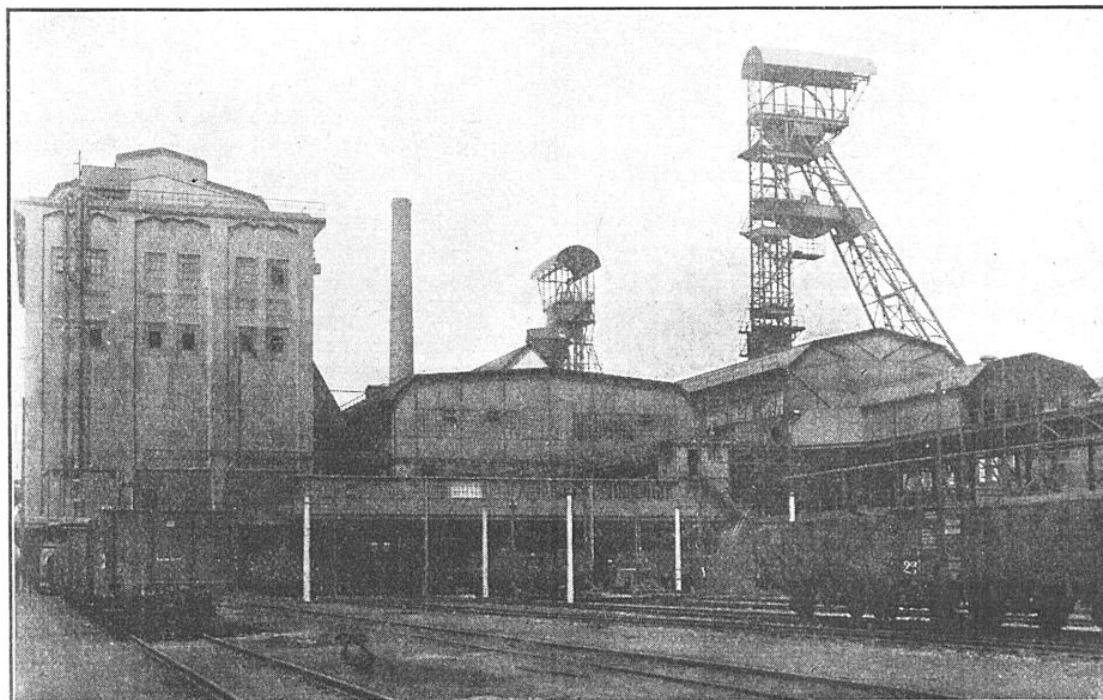
FIG. 2. — LAVOIR POUR L'ÉPURATION DU CHARBON PAR L'INTERMÉDIAIRE DE MILIEUX DENSES, A SOPHIA-JACOBA (BASSIN D'AIX-LA-CHAPELLE)
