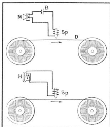
FIG. 2. — ENREGISTREMENT ET REPRODUCTION SUR FIL D'ACIER
