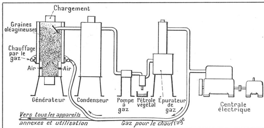
FIG. 3. — SCHÉMA DE FONCTIONNEMENT DE L'USINE CHARLES ROUX
