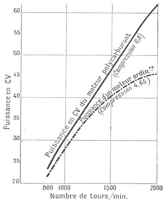
FIG. 8. — GRAPHIQUE MONTRANT LES VARIATIONS DE PUISSANCE DU MOTEUR POLYCARBURANT (TRAIT PLEIN) COMPARÉES A CELLES DU MOTEUR ORDINAIRE (TRAIT POINTILLÉ), EN FONCTION DU NOMBRE DE TOURS
