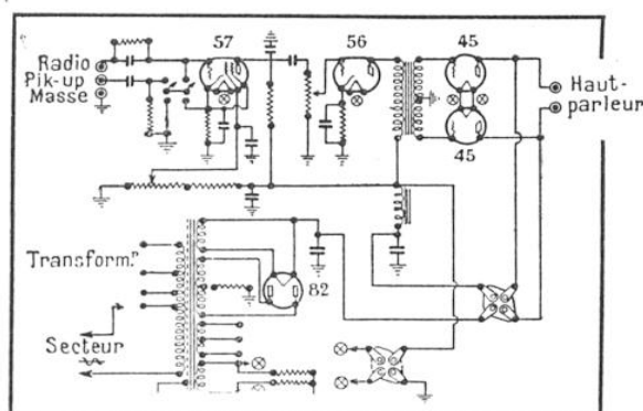
FIG. 5. — SCHÉMA DE L'AMPLIFICATEUR BASSE FRÉQUENCE POUR L'ENREGISTREMENT D'AMATEURS SUR DISQUES
