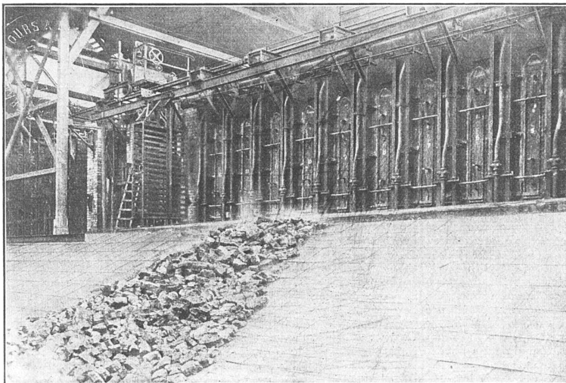
FIG. 3. — ASPECT DU SEMI-COKE OBTENU A PARTIR DE « FINES » (CHARBONS PULVÉRENTS), A LA SORTIE DES FOURS, A LA SOCIÉTÉ DES MINES DE MONTRAMBERT (LOIRE)
