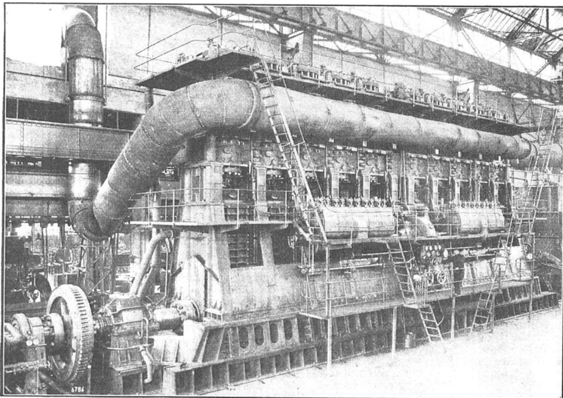
FIG. 1. — LE PLUS GRAND MOTEUR DIESEL MARIN DU MONDE, CONSTRUIT PAR FIAT POUR LE MOTORSHIP ITALIEN « VULCANIA », ET QUI, AUX ESSAIS AU FREIN EFFECTUÉS EN AVRIL DERNIER, A DÉVELOPPÉ UNE PUISSANCE DE PLUS DE 16.500 CHEVAUX
