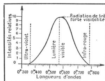
FIG. 3. - RAYONNEMENT D'UNE LAMPE « STELLA-BOULE »
