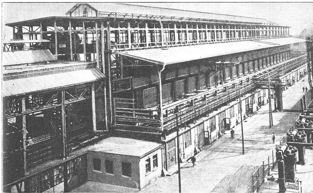
FIG. 4. — LES USINES ALLEMANDES DE LEUNA ONT POUSSÉ TRÈS LOIN L'ÉTUDE DE LA CHIMIE DU CHARBON. ON VOIT ICI LES BATIMENTS OU SE TERMINE, PAR CATALYSE, LA FABRICATION DE L'AMMONIAQUE SYNTHÉTIQUE À PARTIR DE L'HYDROGÈNE DES GAZ DE FOURS À COKE
