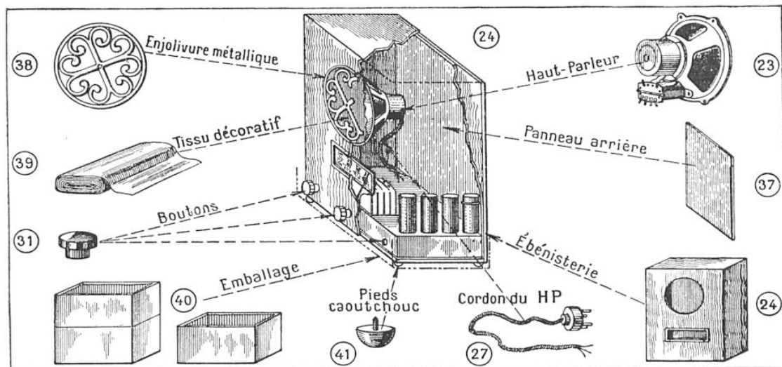
FIG. 2. — ENSEMBLE DU RÉCEPTEUR SUPERHÉTÉRODYNE QUATRE LAMPES ET UNE VALVE Les chiffres entourés d'un cercle correspondent au numérotage des pièces (tableau II).
