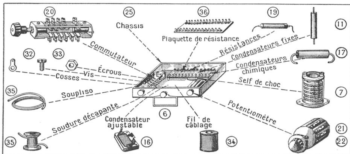
FIG. 4. — LE CHASSIS VU DE DESSOUS DU POSTE RÉCEPTEUR QUATRE LAMPES PLUS UNE VALVE
