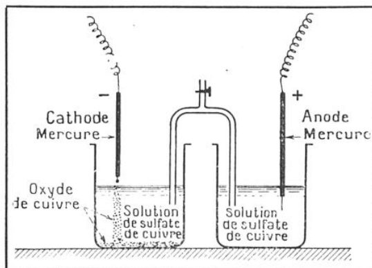
SCHÉMA DU DISPOSITIF D'ÉLECTROLYSE A ARC DE M. JOLIBOIS
