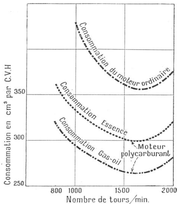
FIG. 9. — CONSOMMATION EN CENTIMÈTRES CUBES, PAR CHEVAL-HEURE, DES DIFFÉRENTS COMBUSTIBLES : 1° DANS LE MOTEUR ORDINAIRE (ESSENCE) ; 2° DANS LE MOTEUR POLYCARBURANT (ESSENCE OU GAS OIL) Le carburant volatil et le carburant lourd sont figurés chacun par une courbe spéciale.
