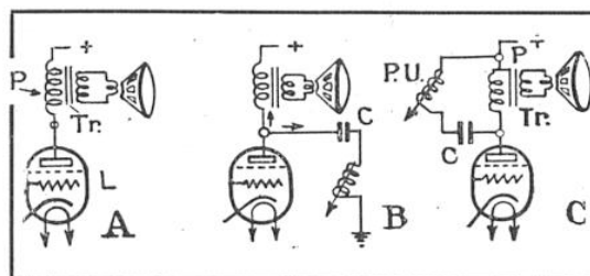
FIG. 10. — SCHÉMA DE MONTAGE MONTRANT COMMENT ON A PU ÉVITER TOUTE DISTORSION PROVOQUÉE PAR LE BRANCHEMENT DU PICK-UP ENREGISTREUR SUR DISQUES
