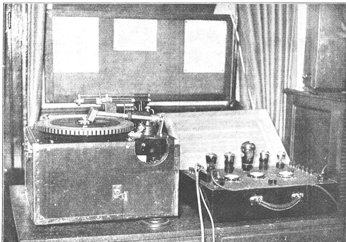
FIG. 1. — ENSEMBLE DU DISPOSITIF D'ENREGISTREMENT ÉLECTROMAGNÉTIQUE SUR DISQUES DES RADIOREPORTAGES INSTALLÉ AU « PETIT PARISIEN »
