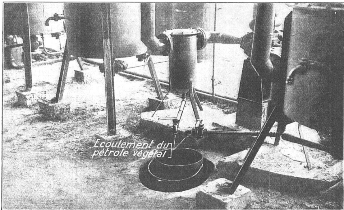
FIG. 2. — LA SORTIE DU PÉTROLE BRUT PRODUIT PAR LA DISTILLATION DES HUILES EXTRAITES DES PLANTES OLÉAGINEUSES DANS L'INSTALLATION CI-DESSUS. Le moteur polycarburant, dont nous parlons plus loin, permet d'utiliser industriellement le «pétrole végétal».
