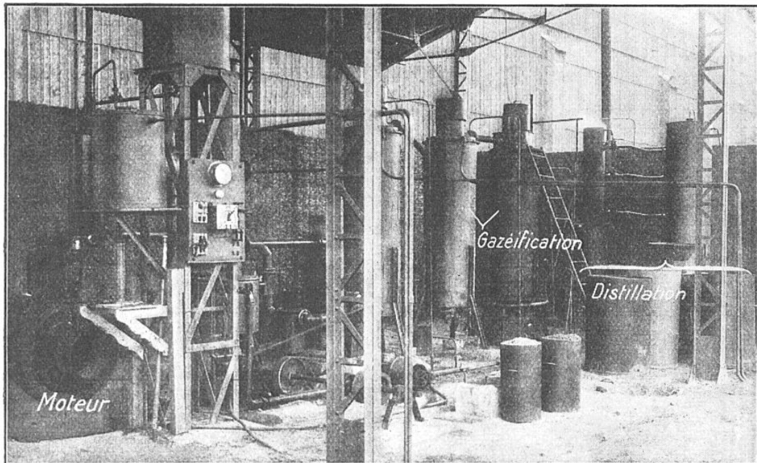
FIG. 1. — L'USINE MOBILE CHARLES ROUX POUR LA PRODUCTION DU CARBURANT COLONIAL. Au premier plan, l'usine de production du pétrole végétal brut (gazéification). Au second, les appareils, distincts, de cracking et de rectification (distillation).
