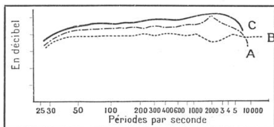
FIG. 9. — EN COMBINANT LES COURBES DE RÉPONSE DU MICROPHONE (A) ET DU TRANSFORMATEUR DE LIAISON (B), ON OBTIENT UNE COURBE C PRESQUE RECTILIGNE
