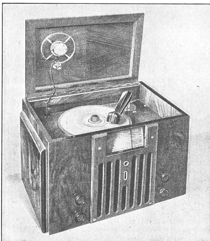
FIG. 8. — L'APPAREIL « SOUBITEZ-77 » (PROCÉDÉS « RETERSON ») PERMETTANT A VOLONTÉ L'ENREGISTREMENT SUR DISQUES ET LA REPRODUCTION
