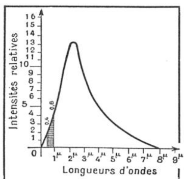
FIG. 2. — RAYONNEMENT DU FILAMENT D'UNE LAMPE A INCANDESCENCE
