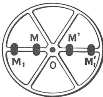
FIG. 1. — L'ÉNERGIE DE ROTATION DE LA TERRE, COMME CELLE D'UN VOLANT, DÉPEND DE LA VITESSE DE ROTATION ET DU MOMENT D'INERTIE
