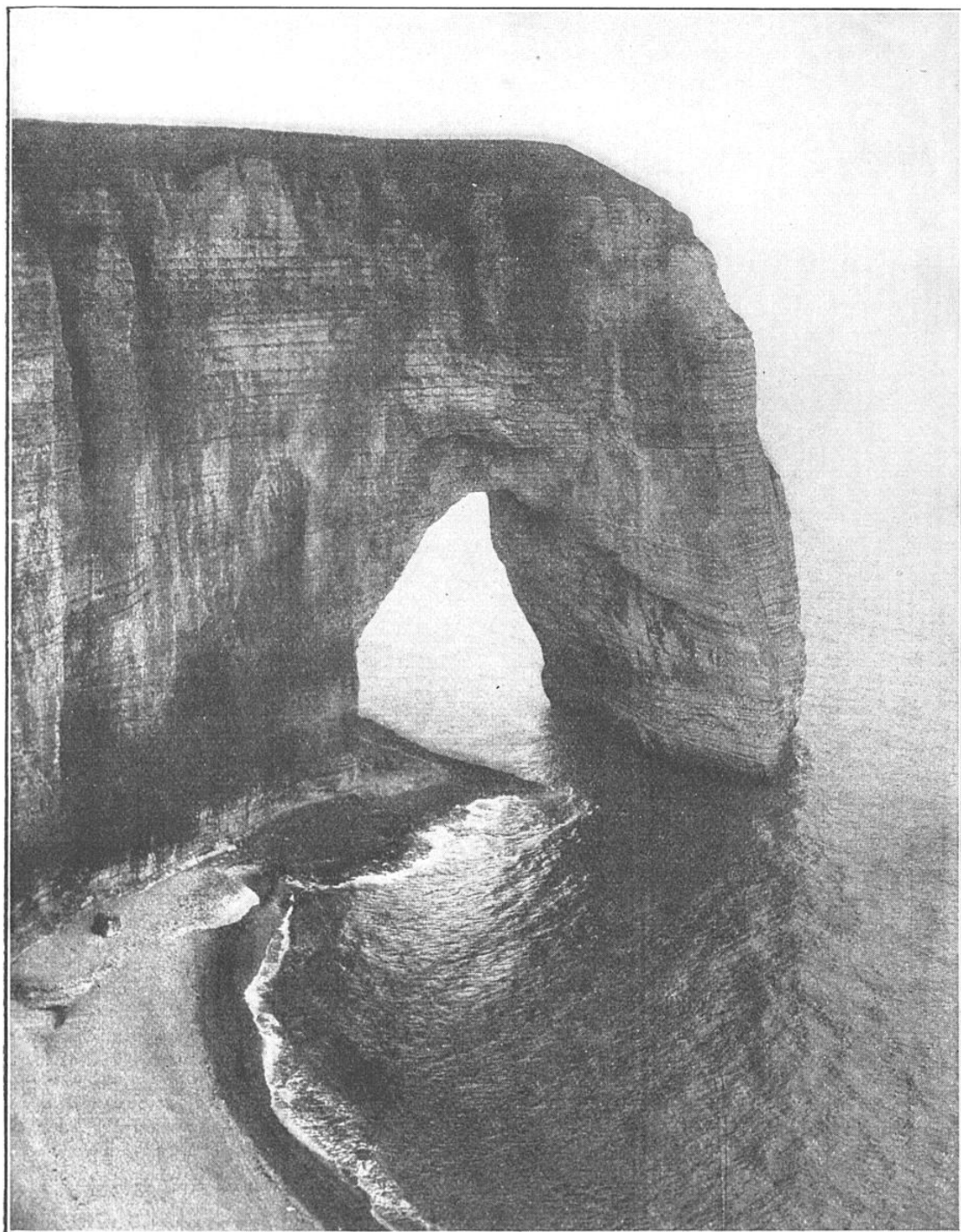
FIG. 3. — L'EFFET PUISSANT DES MARÉES EST MIS EN ÉVIDENCE PAR LA DESTRUCTION PROGRESSIVE DE CERTAINES COTES. ON VOIT ICI LA « MANNEPORTE », DANS LES FALAISES D'ÉTRE-TAT, SUR LES RIVES DE LA MANCHE (SEINE-INFÉRIEURE)
