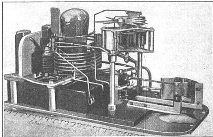
FIG. 7. — MODÈLE ACTUEL DU RADIOÉMETTEUR UTILISÉ POUR LES RADIOSONDAGES ATMOSPHÉRIQUES
