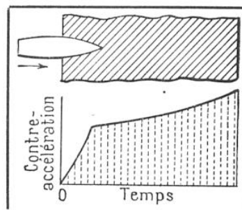
FIG. 4. — CONTRE-ACCÉLÉRATION THÉORIQUE DANS UN BLINDAGE INDÉFINI
