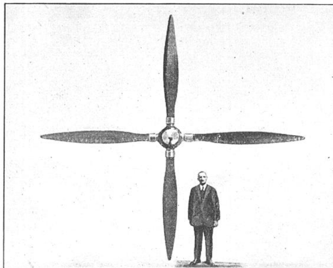
FIG. 1. — LE DIAMÈTRE DE L'HÉLICE DOIT AUGMENTER AU FUR ET À MESURE QUE DIMINUE LA DENSITÉ DU FLUIDE PORTEUR, C'EST-À-DIRE QUAND L'ALTITUDE CROIT. Voici l'hélice prévue par M. Waseige pour le vol à 10.000 mètres.
