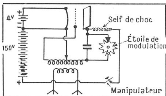
FIG. 8. — SCHÉMA DU RADIOÉMETTEUR QUI ASSURE LA TRANSMISSION AUTOMATIQUE PAR T. S. F. DES INDICATIONS DES APPAREILS EMPORTÉS PAR LE BALLON-SONDE
