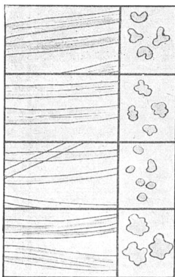
FIG. 4. — MICROGRAPHIES DE FIBRES DE RAYONNE
