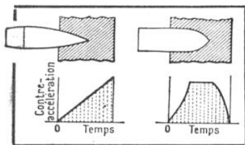
FIG. 3. — GRAPHIQUES MONTRANT, EN BAS, LA CONTRE-ACCÉLÉRATION OPPOSÉE PAR UN BLINDAGE AUX DIFFÉRENTS NIVEAUX DE PÉNÉTRATION, D'APRÈS LA FORME DU PROJECTILE
