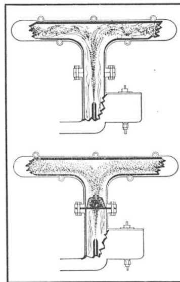
LE TURBO-DIFFUSEUR REND HOMOGÈNE LE MÉLANGE AIR-ESSENCE DANS LA TUYAUTERIE DU MOTEUR
