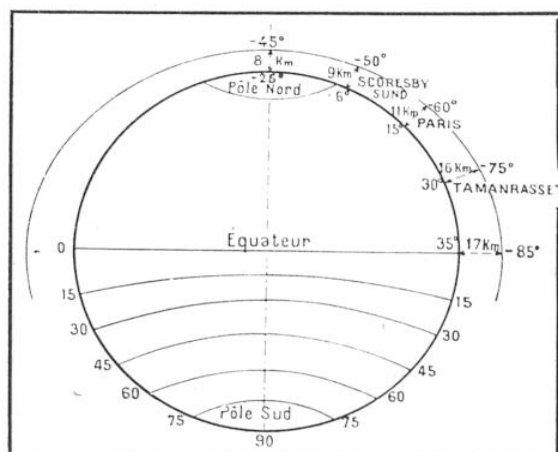
FIG. 2. — TEMPÉRATURES DE LA HAUTE ATMOSPHERE MESURÉES PAR BALLONS-SONDES. C'est au-dessus des régions tropicales et non des pôles que, vers 17 kilomètres d'altitude, on enregistre les températures les plus basses.
