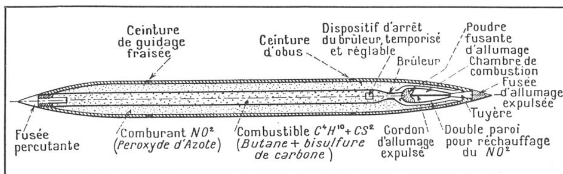
FIG. 6. — UNE FUSÉE « POSSIBLE » SCHÉMATISÉE PAR M. MÉLOT
