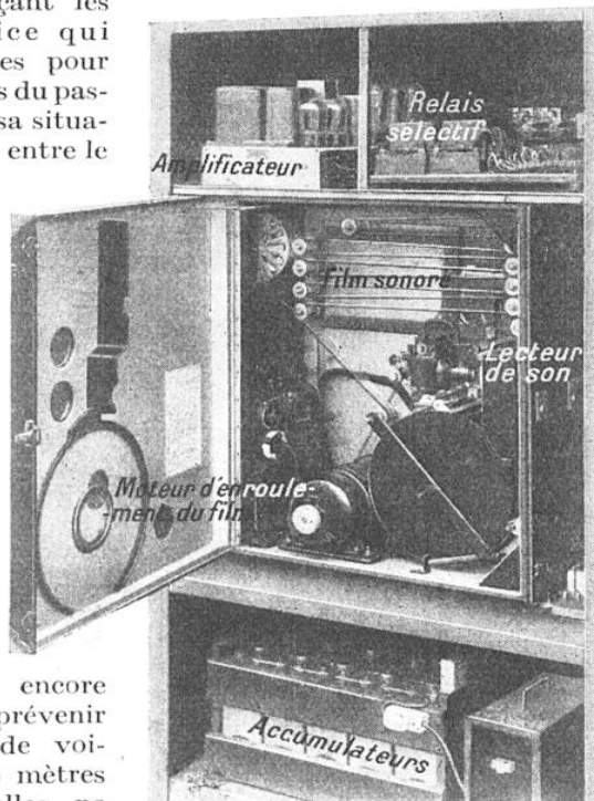
FIG. 3. — ARMOIRE CONTENANT LE MÉCANISME DE COMMANDE DES SIGNAUX SONORES
