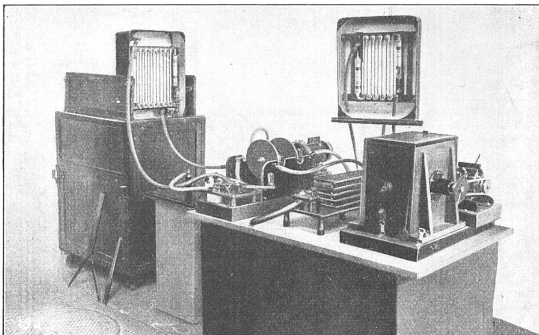
FIG. 4. — CINÉMATOGRAPHIE ULTRA-RAPIDE AVEC LE « STROBORAMA » TYPE A
