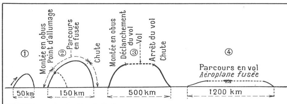
FIG. 5. — LES QUATRE FORMES THÉORIQUES DE LA TRAJECTOIRE DU « TIR » : 1° PAR FUSÉE LIBRE ; 2° PAR OBUS-FUSÉE ; 3° PAR OBUS-FUSÉE VOLANTE ; 4° PAR AVION-FUSÉE Les calculs relatifs à ces tirs sont dus au spécialiste bien connu de nos lecteurs, M. Mélot.
