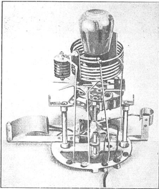
FIG. 6. — RADIOÉMETTEUR EMPORTÉ PAR UN BALLON-SONDE ET EMPLOYÉ POUR LES OBSERVATIONS DE L'« ANNÉE POLAIRE »
