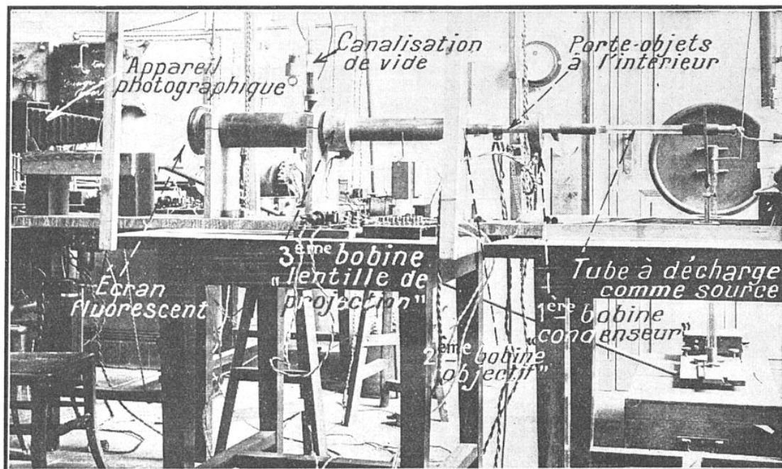
FIG. 3. — VUE D'ENSEMBLE DE L'INSTALLATION DU MICROSCOPE ÉLECTRONIQUE
