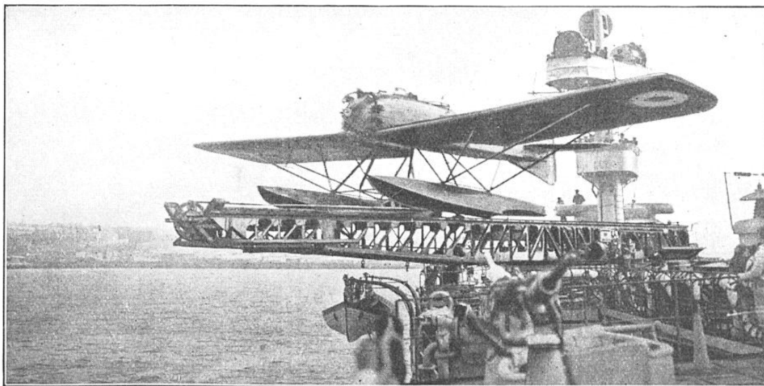
FIG. 3. — LANCEMENT PAR CATAPULTE D'UN HYDRAVION A BORD DU CROISSEUR FRANÇAIS DE 10.000 TONNES « DUQUESNE », QUI POSSÈDE DEUX HYDRAVIONS
