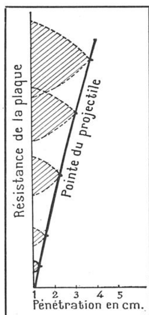
FIG. 1. — GRAPHIQUE CLASSIQUE DE LA PÉNÉTRATION (CENTIMÈTRES) D'UN PROJECTILE DANS UN BLINDAGE EN FONCTION DE LA RÉSISTANCE (EN ORDONNÉE)
