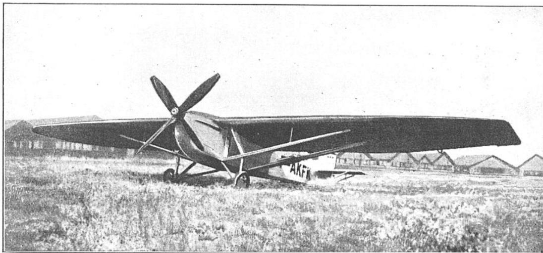
FIG. 2. — L'AVION STRATOSPHERIQUE A CABINE ETANCHE « FARMAN »
