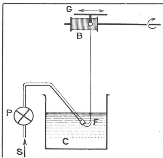
FIG. 2. — SCHÉMA SIMPLIFIÉ D'UNE MACHINE À FILER LA RAYONNE
