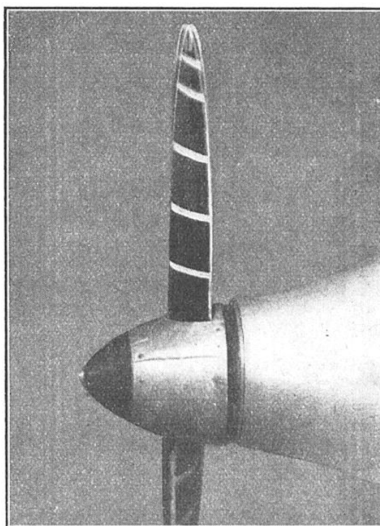
FIG. 3. — MESURE DES FLEXIONS D'UNE HÉLICE PAR LA SUPERPOSITION DE DEUX PHOTOGRAPHIES AU MILLIONIÈME DE SECONDE. Les photos correspondent à des vitesses de l'hélice de 250 à 2.400 tours-minute. Les vitesses correspondantes de l'extrémité de la pale sont, dans les deux cas, de 22 et 216 mètres-seconde.
