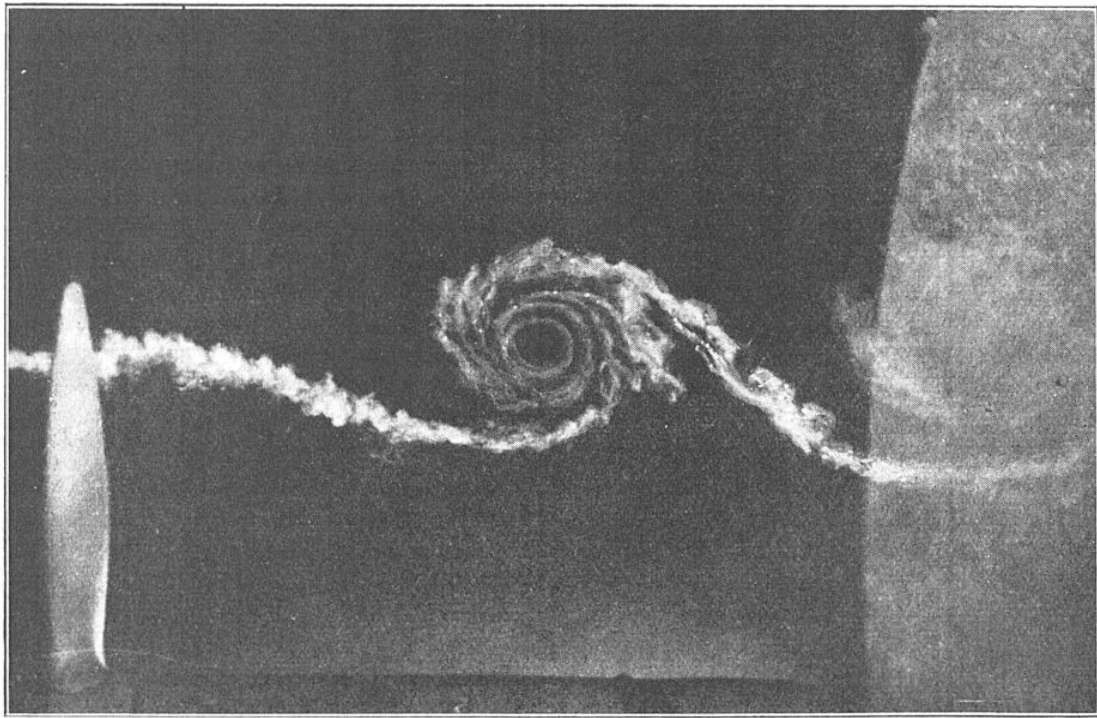
FIG. 1. — PHOTOGRAPHIE AU MILLIONIÈME DE SECONDE DES REMOUS TOURBILLONNAIRES PRODUITS SUR UN JET DE FUMÉE DERRIÈRE UNE HÉLICE (QUE L'ON VOIT À GAUCHE) EN ROTATION RAPIDE DANS UNE SOUFFLERIE (INSTITUT DE MÉCANIQUE DES FLUIDES DE MARSEILLE)
