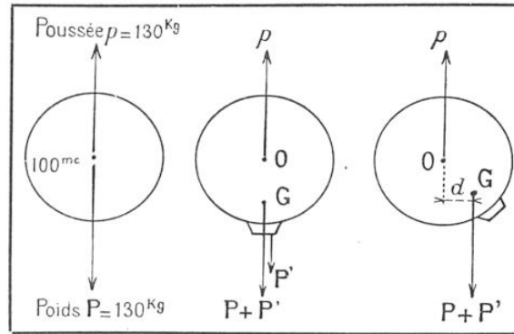
FIG. 1. — SCHÉMA DE PRINCIPE DU STABILISATEUR A BALLONNET D'AIR
