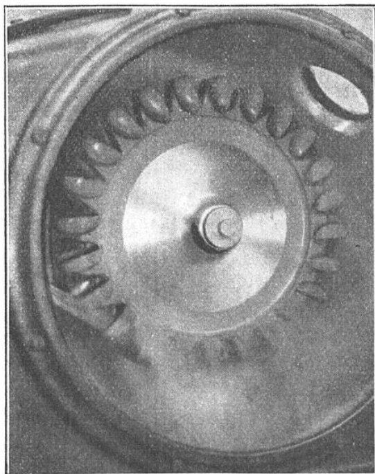
FIG. 2. - ROUE « PELTON » PHOTOGRAPHIÉE EN ARRÊT APPARENT, GRACE A LA STROBOSCOPIE
