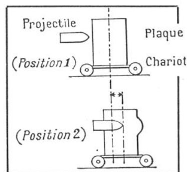
FIG. 2. — LA RÉPARTITION THÉORIQUE DE L'ÉNERGIE DANS LA PERFORATION D'UN BLINDAGE
