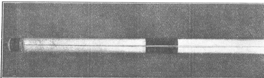
FIG. 6. — MESURE DE LA FLEXION D'UN ARBRE DE CARDAN D'AUTOMOBILE PAR LA SUPERPOSITION DE DEUX PHOTOGRAPHIES AU MILLIONIÈME DE SECONDE
