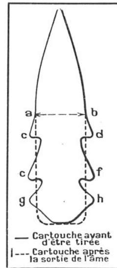
FIG. 7. — LA BALLE GEHRLICH
