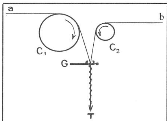
FIG. 10. — SCHÉMA DU PRINCIPE DE LA FABRICATION DES FILS BOUCLÉS
