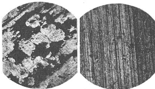
MICROGRAPHIES (GROSSISSEMENT 150 DIAMÈTRES) MONTRANT NETTEMENT LA DIFFÉRENCE DE LA SURFACE D'UN FRAGMENT DE MOTEUR DIESEL AVANT ET APRÈS GRAPHOÏLAGE
