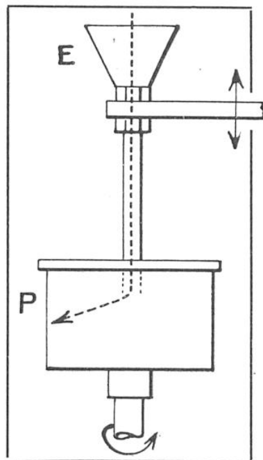
FIG. 3. — L'ENTONNOIR ET LE POT « TOPHAM »
