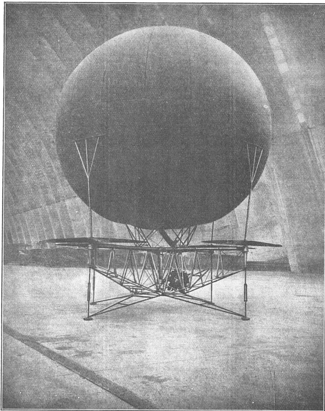
MODÈLE D'ESSAI D'UN HÉLICOSTAT OEHMICHEN, QUI A EFFECTUÉ RÉCEMMENT PLUSIEURS VOIS CONCLUANTS A L'AÉRODROME D'ORLY (SEINE-ET-OISE)
