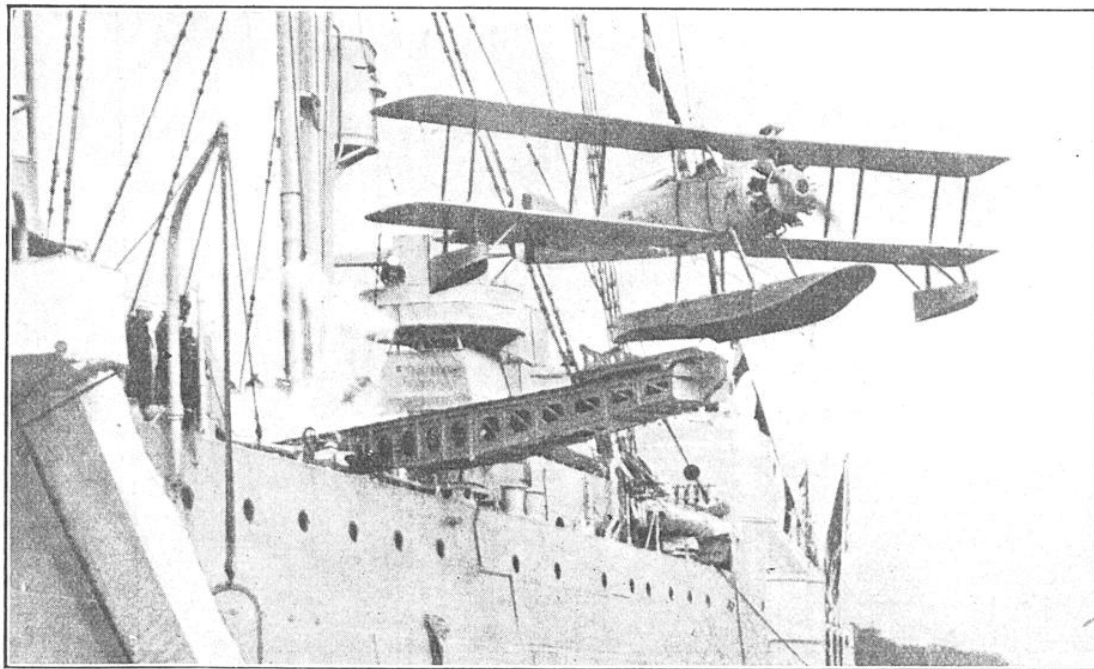
FIG. 1. — CATAPULTAGE « A POUDRE » D'UN HYDRAVION A BORD D'UN CROISEUR AMÉRICAIN C'est en 1921 que le capitaine de frégate américain Hamlet suggéra le remplacement de l'air comprimé, comme « moteur » du chariot de la catapulte, par une charge de poudre. Ce procédé fut expérimenté avec succès en 1923 à bord du superdreadnought de 33.000 tonnes Mississippi .
