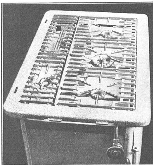
VUE DU DESSUS DE LA « GAZINIÈRE » Au premier plan, le thermostat de réglage.
