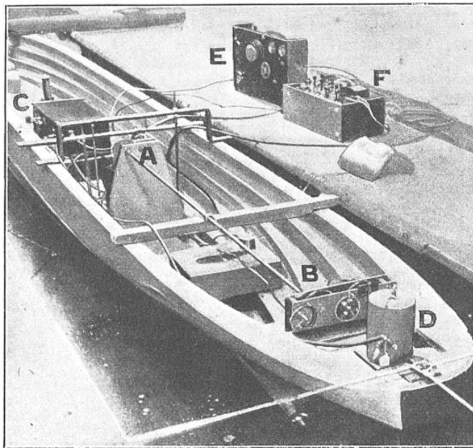
FIG. 4. — VOICI UN MODÈLE RÉDUIT DE NAVIRE ÉQUIPÉ POUR LES ESSAIS CONCERNANT LES VIBRATIONS SUIVANT LA TECHNIQUE DU PROFESSEUR FRANK-M. LEWIS, DE L'INSTITUT D'ARCHITECTURE NAVALE DE NEW YORK
