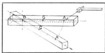
FIG. 1. — DÉFINITION DE L'AXE DE PERCUSSION
