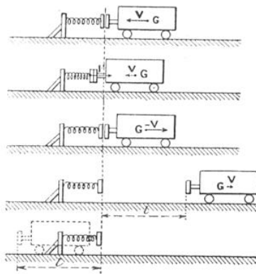
FIG. 5. — UN RESSORT NE PRODUIT PAS D'AMORTISSEMENT Le wagon, arrivant avec la vitesse V , comprime le ressort du butoir ; puis, sous l'action du ressort, repart avec une vitesse égale et de sens contraire.
