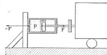
FIG. 6. — BUTOIR AVEC DISPOSITIF D'AMORTISSEMENT
