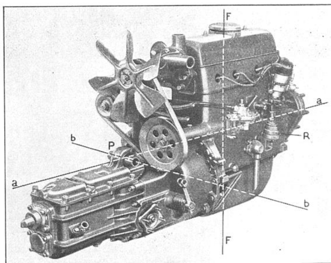
FIG. 12. — LE MOTEUR D'AUTOMOBILE ET LES AXES AUTOUR DESQUELS IL PEUT OSCILLER DANS LE MONTAGE « PAUSODYNE »
