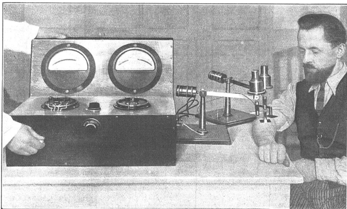
FIG. 2. — MESURE DE LA RÉSISTANCE ÉLECTRIQUE DE L'ÉPIDERME D'UN OUVRIER Cette résistance constitue un coefficient important contre le danger d'électrocution.
