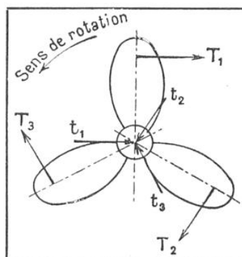
FIG. 1. — LES IRRÉGULARITÉS EXISTANT ENTRE LES PALES D'UNE HÉLICE PEUVENT ÊTRE UNE GRAVE SOURCE DE VIBRATIONS T_1 , T_2 et T_3 sont les réactions tangentielles qui s'exercent sur les trois pales. Si elles ont des valeurs différentes, les trois forces t_1 , t_2 et t_3 , qui leur sont égales, ne se font pas équilibre et l'axe se trouve sollicité par une force tournante qui, par l'intermédiaire des paliers, engendre des vibrations importantes dans la charpente et la coque du navire.
