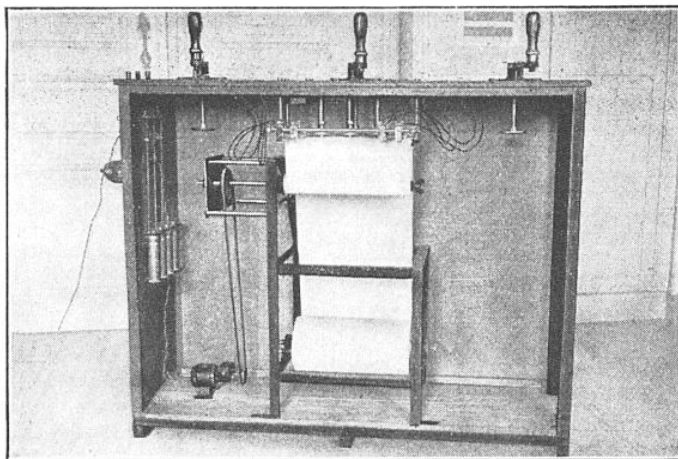
FIG. 11. — L'« AUTOMATOGRAPHE » SOLLIER-DRABS UTILISÉ A L'INSTITUT DE BRUXELLES
