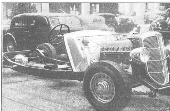
FIG. 3. — VUE D'ENSEMBLE DE LA NOUVELLE 6 CYLINDRES « UNIC », DONT LE MOTEUR A SOUPAPES EN TÊTE COMPORTE DE NOMBREUX CARTERS ET LA CULASSE EN ALLIAGE D'ALUMINIUM
