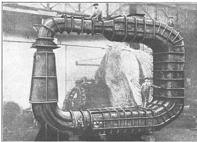
FIG. 5. — TUNNEL HYDRODYNAMIQUE POUR L'ÉTUDE DE LA CAVITATION AU LABORATOIRE WILLIAM FROUDE, DE TEDDINGTON (GRANDE-BRETAGNE)
