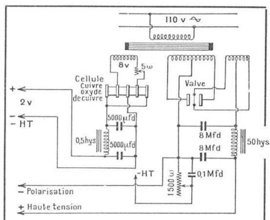
FIG. 2. — ALIMENTATION D'UN POSTE A LAMPES A CHAUFFAGE DIRECT SUR UN SECTEUR A COURANT ALTERNATIF
