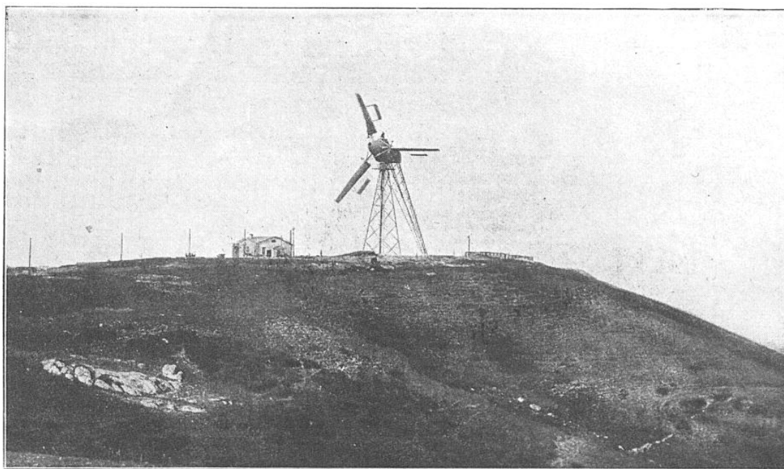
FIG. 4. — ENSEMBLE DE LA STATION ÉOLIENNE DE 100 KW DE BALACLAVA (CRIMÉE) Les petites pales visibles à côté des grandes règlent automatiquement la vitesse de l'éolienne à 30 t/mn
