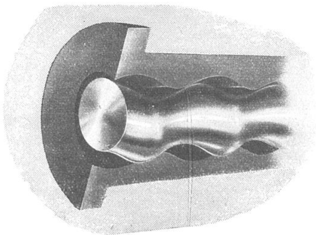
INTÉRIEUR DE LA POMPE P. C. M.
