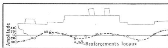
FIG. 3. — VOICI UN EXEMPLE D'UNE COURBE ÉLASTIQUE RELEVÉE À L'OSCILLOGRAPHIE SUR UN NAVIRE DE 180 MÈTRES DE LONG
