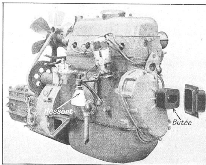
FIG. 14. — LES MOUVEMENTS BRUSQUES PROVOQUÉS PAR LES INÉGALITÉS DE LA ROUTE SONT LIMITÉS PAR UNE BUTÉE SPÉCIALE EN CAOUTCHOUC
