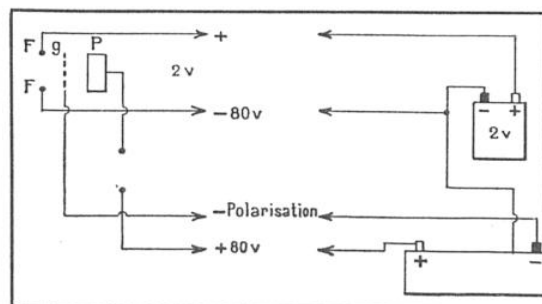
FIG. 1. — ALIMENTATION D'UN POSTE SUR BATTERIES D'ACCUMULATEURS
