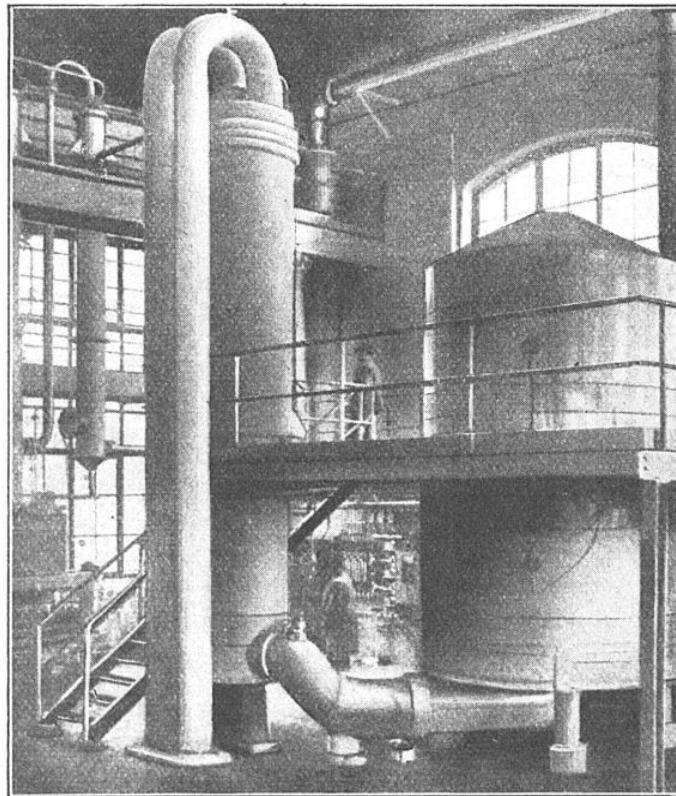
VUE PARTIELLE DE L'APPAREILLAGE SERVANT A LA FABRICATION DU BUTADIÈNE, DONT LA POLYMERISATION DONNE LE CAOUTCHOUC SYNTHÉTIQUE « BUNA », AUX USINES DE L'« I. G. FARBEINDUSTRIE » (ALLEMAGNE)
