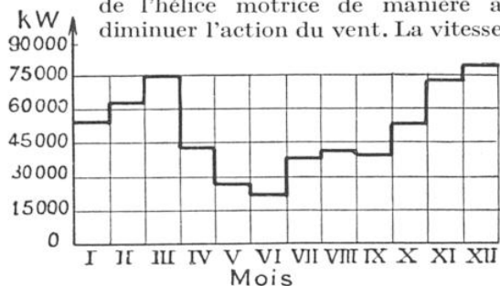
FIG. 2. — GRAPHIQUE DES VARIATIONS DE L'ÉNERGIE FOURNIE AU COURS D'UNE ANNÉE PAR LA STATION ÉOLIENNE D'ESSAIS DE BALACLAVA (U. R. S. S.)
