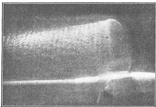
FIG. 6. — LA PRÉCAVITATION D'UNE HÉLICE PHOTOGRAPHIÉE AU TUNNEL HYDRODYNAMIQUE DE HAMBOURG (ALLEMAGNE)
