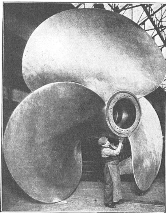
FIG. 10. — VOICI UNE DES HÉLICES PRIMITIVES A TROIS PALES DU PAQUEBOT « NORMANDIE »
