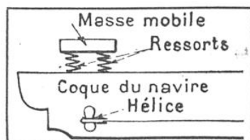
FIG. 8. — SCHÉMA DE PRINCIPE DE L'ABSORBEUR DYNAMIQUE DE VIBRATIONS SUIVANT LE SYSTÈME « FRAHM »
