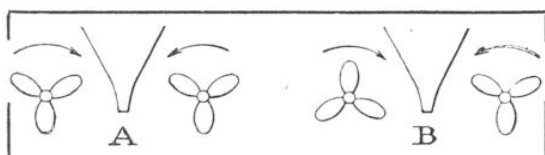
FIG. 2. — LES DEUX HÉLICES DE GAUCHE SONT DITES « EN PHASE » ; CELLES DE DROITE, AU CONTRAIRE, SONT DITES « EN OPPOSITION » On voit facilement que, puisque ces deux dernières hélices tournent en sens inverse, deux de leurs pales passent au même instant par l'horizontale.
