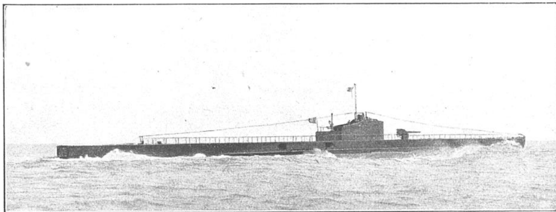
FIG. 5. — LE SOUS-MARIN FRANÇAIS « AGOSTA ». Son déplacement est de 1 379 tonnes en surface et de 2 060 tonnes en plongée. Sa vitesse, en surface, atteint 18 nœuds ; en plongée, 10 nœuds. Son armement comprend 1 canon de 100 mm, 1 canon de 37 mm, 1 mitrailleuse, 11 tubes lance-torpilles de 550 mm. L'Agosta a été lancé en 1934.
