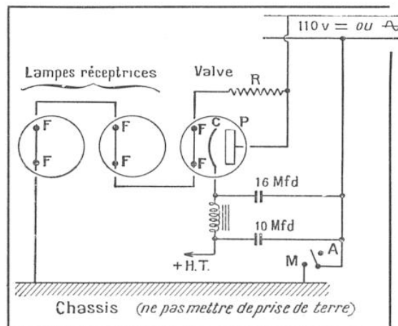
FIG. 5. — ALIMENTATION D'UN POSTE TOUTS COURANTS (ALTERNATIF OU CONTINU)
