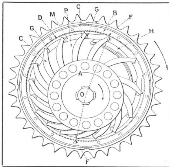
SCHÉMA DU CHANGEMENT DE VITESSE PROGRESSIF « MILPAT » A DOUZE VITESSES
