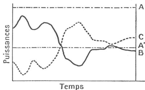
FIG. 1. — COURBES DU TRAVAIL EN PARALLÈLE D'UNE STATION ÉOLIENNE ET D'UNE CENTRALE HYDRAULIQUE
