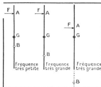
FIG. 3. — L'AXE D'OSCILLATION SE DÉPLACE VERS LE BAS, LORSQUE LA FRÉQUENCE DE LA FORCE F AUGMENTE
