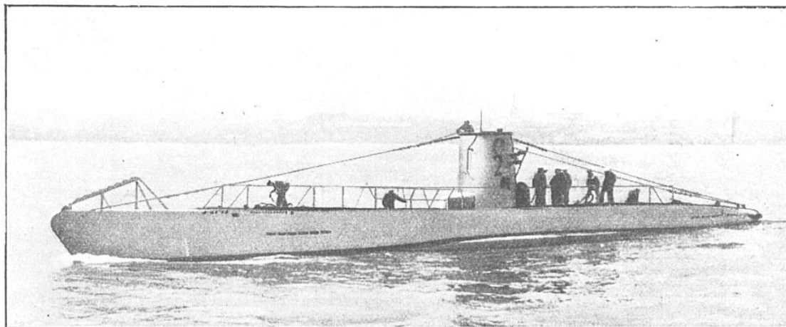
FIG. 2. — VOICI LE NOUVEAU SOUS-MARIN ALLEMAND DE PETIT TONNAGE (250 TONNES) La vitesse de ces bâtiments atteint 15 nœuds en surface et 8 nœuds en plongée. Leur rayon d'action est de 5 600 km. Ils portent 3 tubes lance-torpilles et un approvisionnement de 9 torpilles
