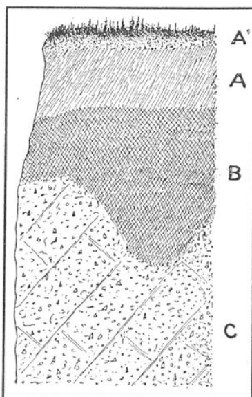
FIG. 1. — COUPE SCHÉMATIQUE D'UN SOL FORMÉ SUR LE GRANULITE (SAINT-YRIEIX-LE-DEJOLAT, CORRÈZE)
