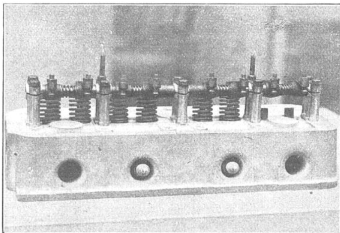
FIG. 2. — CULASSE EN ALLIAGE D'ALUMINIUM « SPEED » POUR MOTEUR 11 CH DE VOITURE CITROËN A TRACTION AVANT
