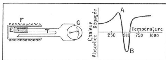
FIG. 3. — L'ANALYSE THERMIQUE D'UN SOL. L'échantillon E est chauffé au four électrique F, cependant qu'on mesure, à l'aide du couple thermoelectrique T, la différence de température entre le four et l'échantillon. La courbe ainsi tracée montre en A un dégagement, et en B une absorption de chaleur.
