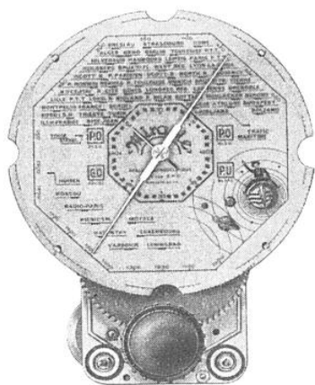
LE CADRAN GYROSCOPIQUE
