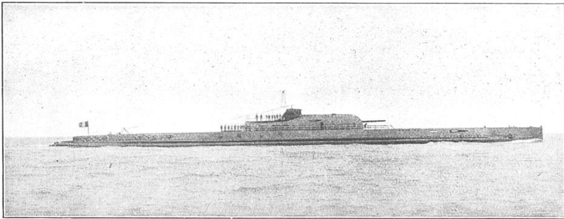
FIG. 4. — LE « SURCOUF », SOUS-MARIN DE CROISIÈRE FRANÇAIS LE PLUS GRAND DU MONDE. Construite en 1927, entrée en service en 1934, cette unité a un déplacement de 2 926 tonnes. Sa vitesse, en surface, est de 18 nœuds et, en plongée, de 10 nœuds. Son rayon d'action est de 12 000 milles à 10 nœuds. Elle est armée de 2 canons de 203 mm, 2 canons de 37 mm, 4 mitrailleuses et 10 tubes lance-torpilles de 550 mm. Son équipage est de 150 hommes. Le Surcouf est entré en service en 1934.
