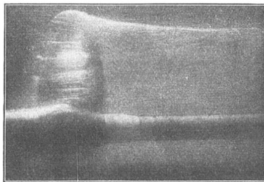
FIG. 7. — LA CAVITATION D'UNE HÉLICE TELLE QU'ON L'OBSERVE AU TUNNEL HYDRODYNAMIQUE DE HAMBOURG
