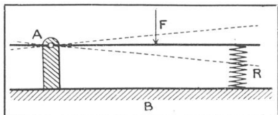
FIG. 7. — BARRE HORIZONTALE, ARTICULÉE EN A ET SUPPORTÉE PAR UN RESSORT R , SOUMISE A UNE FORCE PÉRIODIQUE F La barre oscille sous l'action de la force périodique F en comprimant ou en étirant le ressort.
