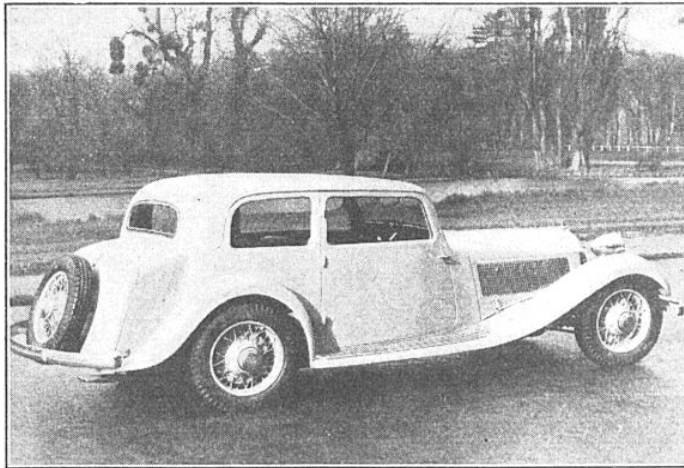
FIG. 1. — CETTE « BABY SPORT » TALBOT EST ENTIÈREMENT CARROSSÉE EN TOLE D'ALLIAGE D'ALUMINIUM
