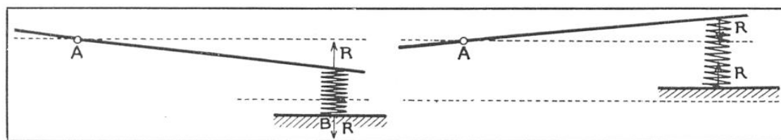
FIG. 9. — COMMENT SE PRODUISENT LES TRÉPIDATIONS D'UNE VOITURE AUTOMOBILE
