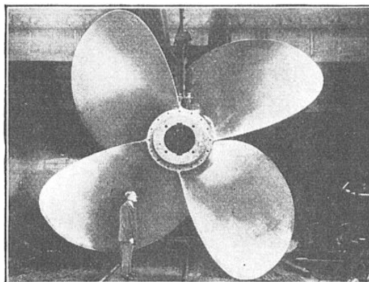
FIG. 9. — VOICI UNE HÉLICE DE LA « QUEEN MARY » QUI VIENT DE PRENDRE LA MER. Cette hélice a 6 m de diamètre et pèse 35,5 tonnes. Son poids brut de fonderie était de 54 tonnes.
