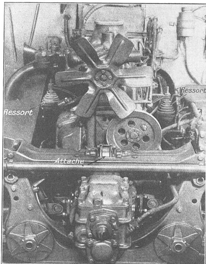
FIG. 13. — VUE AVANT D'UN MOTEUR MONTÉ SUR LE CHÂSSIS PAR LE DISPOSITIF « PAUSODYNE »
