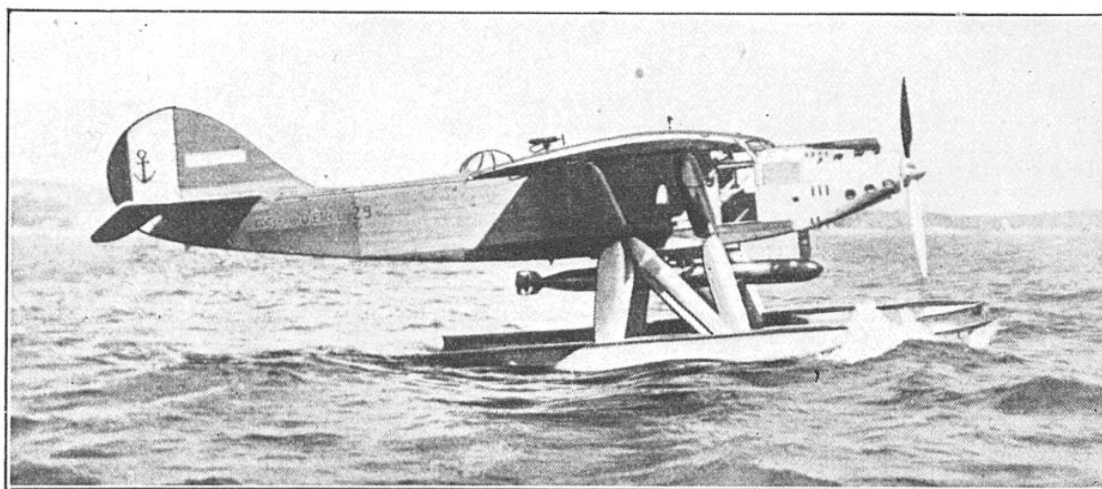
FIG. 12. — L'HYDRAVION TORPILLEUR FRANÇAIS « LATÉCOÈRE 29-0 » (650 CH, VITESSE MAXIMUM AU NIVEAU DE LA MER 230 KM/H, PEUT EMPORTER UNE TORPILLE DE 450 MM
