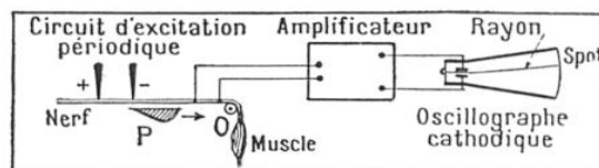
FIG. 6. — SCHÉMA EXPLIQUANT LE FONCTIONNEMENT DE L'APPAREILLAGE CI-DESSUS
