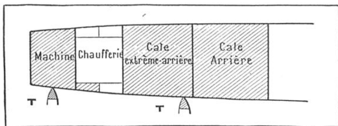
FIG. 2. — COUPE HORIZONTALE SCHÉMATIQUE SOUS LA FLOT- TAISON D'UN CARGO A MACHINE ARRIÈRE
