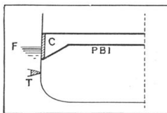
FIG. 9. — COUPE AU MAITRE-COUPLE D'UN CUIRASSÉ SANS PROTECTION SOUS-MARINE. La torpille explosant en T, sous l'effet de bourrage de l'eau, produit des dégâts graves à l'intérieur du navire et peut disloquer la cuirasse de ceinture C et le pont blindé inférieur PBI. Une torpille à faible charge, atteignant la flottaison, ne fera aucun dégât, tout comme un obus éclatant sur la ceinture sans la perforer.
