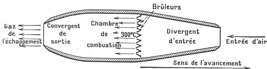
FIG. 7. — SCHÉMA DE PRINCIPE PERMETTANT DE COMPRENDRE AISÉMENT LE FONCTIONNEMENT DE LA TUYÈRE THERMOPROPULSIVE « LEDUC-BREGUET »
