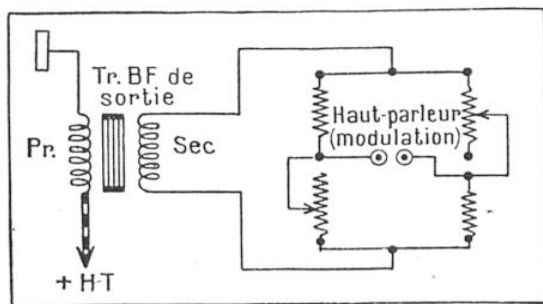
FIG. 1. — SCHÉMA D'UN CIRCUIT EXPENSEUR
