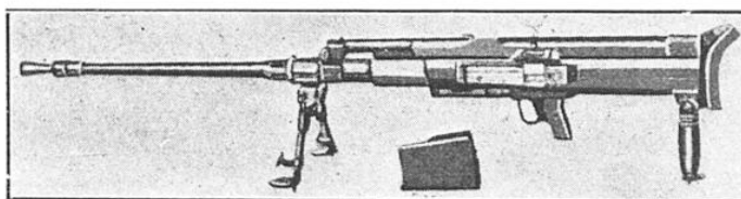
FIG. 5. — CETTE ARME PORTATIVE ANTICHARS, DE FABRICATION SUISSE, A UNE ACTION EFFICACE CONTRE LES ENGINS BLINDÉS JUSQU'À UNE DISTANCE MAXIMUM DE 500 M. Le calibre de cette arme est de 2 cm et la présence d'un frein de bouche rend son recul supportable pour l'épaule du tireur. L'obus de rupture, qui pèse 140 gr, a une vitesse initiale de 750 m/sec et peut perforer une plaque de blindage de 25 mm à 500 m de distance.
