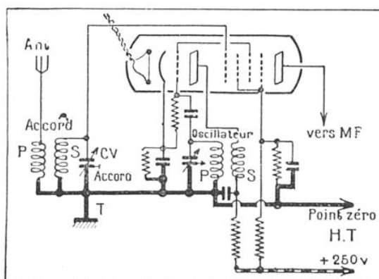
FIG. 4. — MONTAGE D'UNE TRIODE-HEXODE SUR LES BOBINAGES ACCORD ET MODULATEUR
