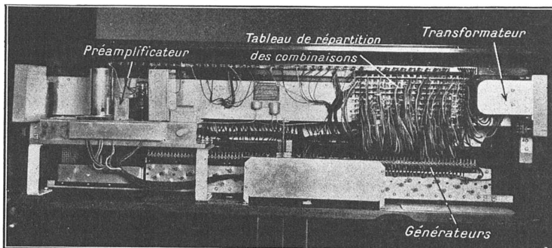
FIG. 6. — L'INTÉRIEUR DE L'ORGUE « HAMMOND »
