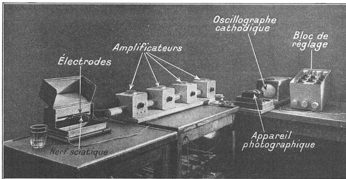
FIG. 5. — L'APPAREILLAGE RADIOÉLECTRIQUE MONTÉ AU LABORATOIRE DE PHYSIOLOGIE DE LA SORBONNE POUR LA MESURE DE L'INFLUX NERVEUX
