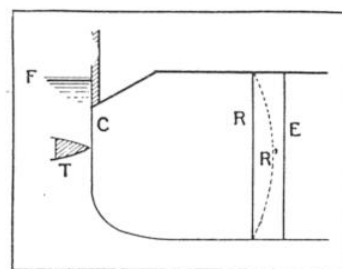
FIG. 3. — COUPE TRANSVERSALE SCHÉMATIQUE D'UN CAISSON DE PROTECTION SOUS-MARINE DU TYPE AL- LEMAND
