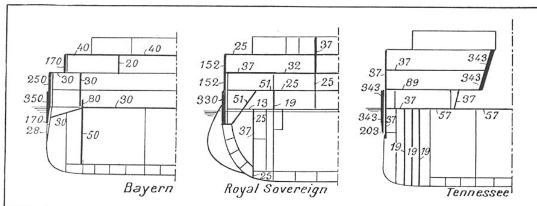
FIG. 4, 5 ET 6. — QUELQUES EXEMPLES DE PROTECTION SOUS-MARINE
