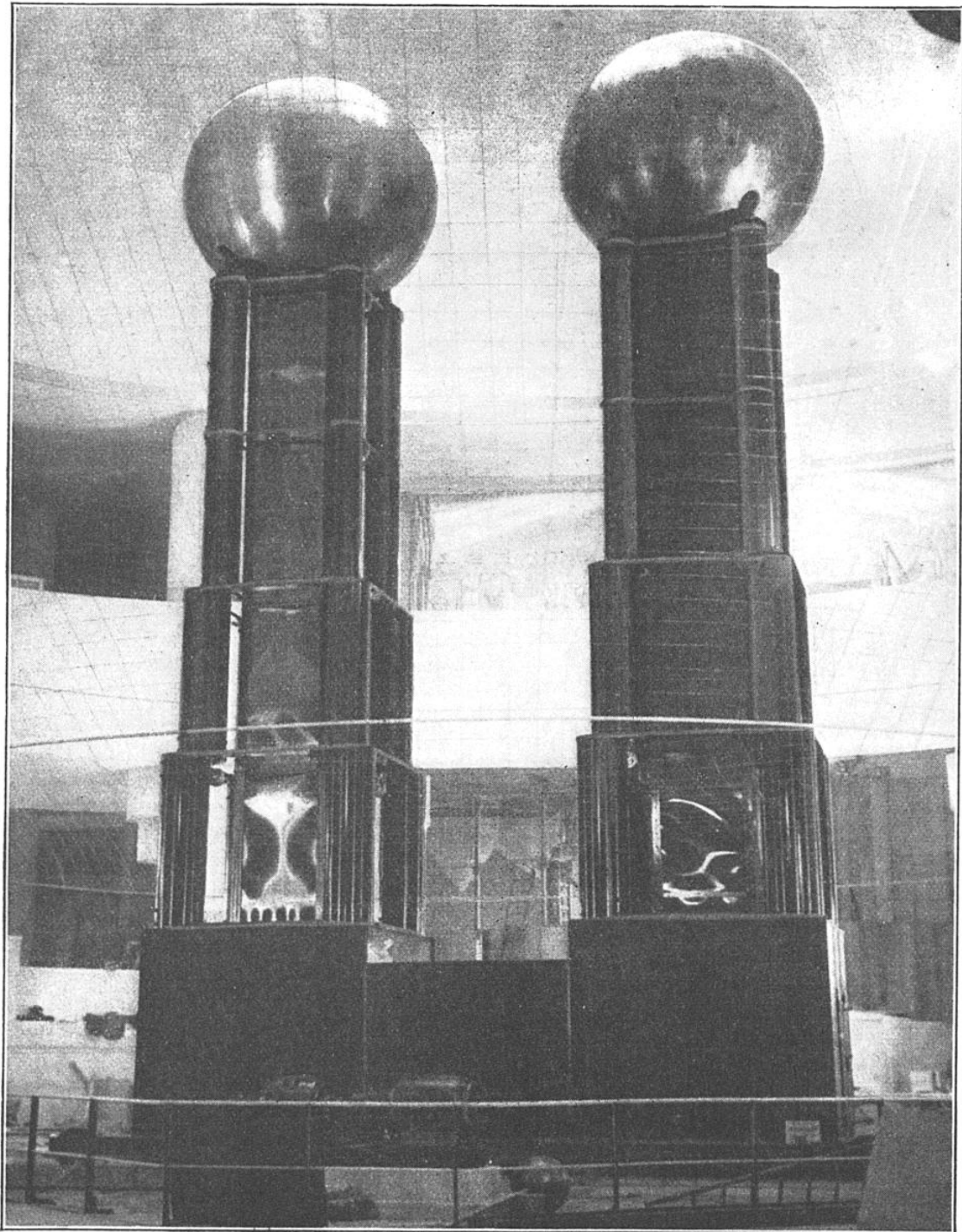
VOICI LA MACHINE ÉLECTROSTATIQUE A 3 MILLIONS DE VOLTS DU PALAIS DE LA DÉCOUVERTE Chaque sphère creuse de 3 m de diamètre en laiton poli est chargée à plus de deux millions de volts, l'une positivement, l'autre négativement, par l'accumulation de charges élémentaires. Chaque sphère, de 1 500 kg, est supportée par des pylônes en bakélite de 9 m de haut reposant eux-mêmes sur une chambre de 2 m 60 de haut. On remarque le filet métallique protecteur de 20 m de diamètre formant cage de Faraday.
