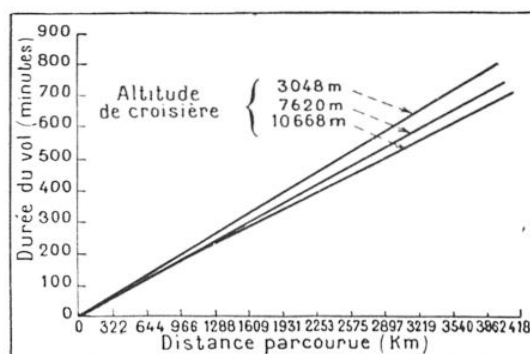
FIG. 6. — LE RAYON D'ACTION DU VOYAGE AÉRIEN NE CROIT PAS SENSIBLEMENT AVEC L'ALTITUDE A LAQUELLE IL S'EFFECTUE. Par contre, c'est la rapidité du voyage qui augmente, la résistance de l'air étant plus faible. Le bénéfice du voyage stratosphérique consiste donc dans la vitesse, non dans la distance parcourue.
