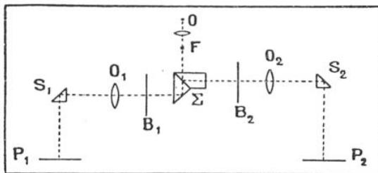
FIG. 6. — SCHÉMA DU « BLINK MICROSCOPE » P_1 P_2 , clichés à comparer ; S_1 S_2 , prismes à réflexion totale ; O_1 O_2 , objectifs ; \Sigma , deux prismes accolés dont on peut masquer alternativement les faces au moyen des écrans B_1 B_2 ; O , observateur.
