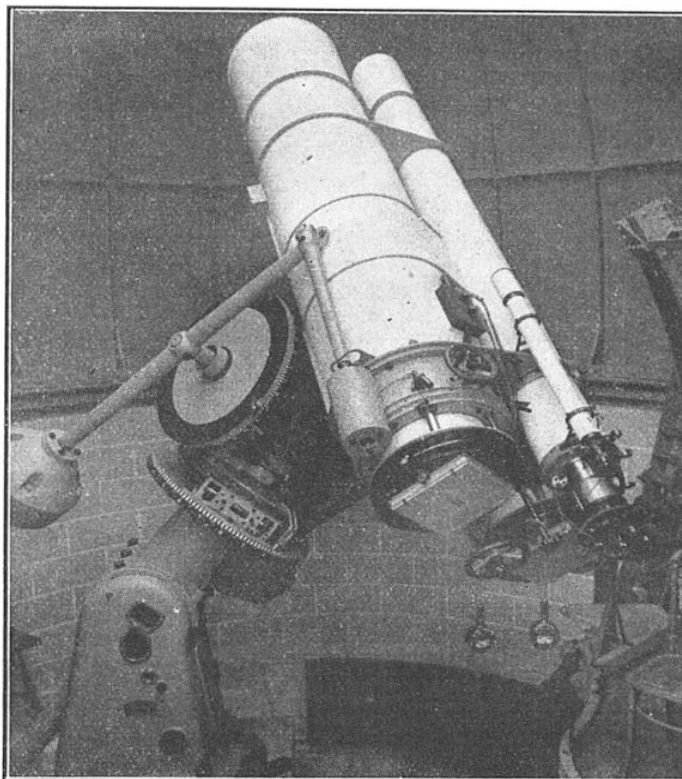
FIG. 3. — VUE GÉNÉRALE DE L'ASTROGRAPHE DOUBLE
