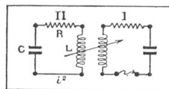
FIG. 10. — SCHÉMA CLASSIQUE DE LA « RÉSONANCE » ENTRE DEUX « CIRCUITS OSCILLANTS » HERTZIENS
