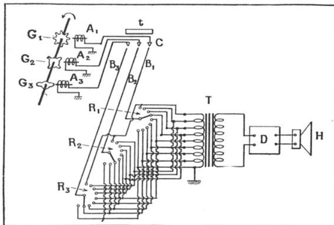
FIG. 4. — SCHÉMA DE PRINCIPE DE L'ORGUE «HAMMOND»
