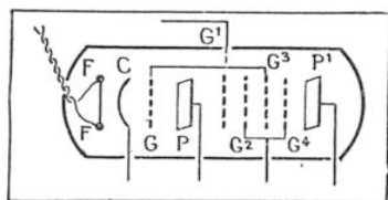
FIG. 3. — SCHÉMA DE LA TRIODE-HEXODE
