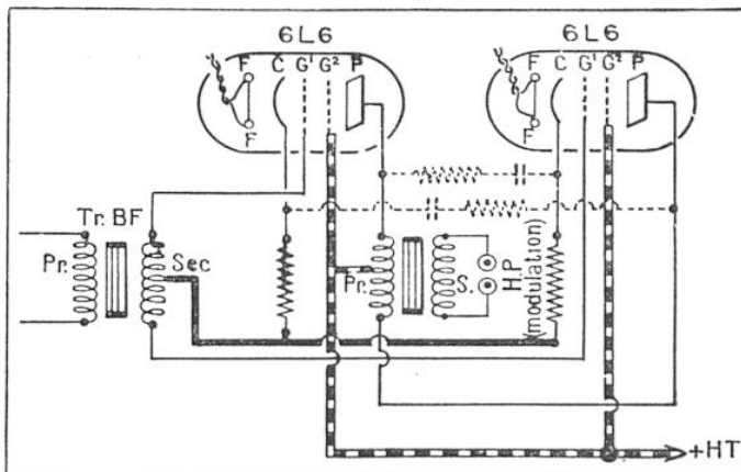
FIG. 2. — SCHÉMA D'UN MONTAGE A CONTRE-RÉACTION EMPLOYÉ AVEC DEUX LAMPES 6-L-6
