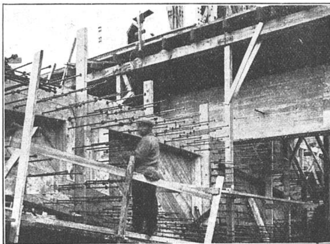
FIG. 2. — VOICI EN COURS DE MONTAGE UNE POUTRE FORMÉE DE PLANCHES RÉUNIES AU MOYEN DE BOULONS
