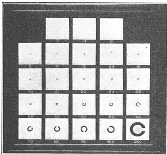
FIG. 1. — LES ANNEAUX DE LANDOLT
