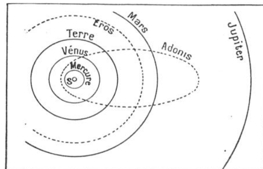
FIG. 8. — TRACÉ DES ORBITES DES PLANÈTES QUI GRAVITENT AUTOUR DU SOLEIL S
