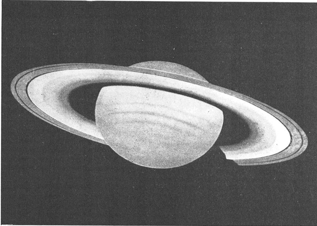
FIG. 1. — ON ADMET AUJOURD'HUI QUE L'ANNEAU DE SATURNE EST FORMÉ PAR L'ENSEMBLE DES TRAJECTOIRES D'INNUMÉRABLES CORPS CÉLESTES DONT LES DIMENSIONS S'ÉCHELONNENT DE QUELQUES CENTIMÈTRES À CELLES DE GRAINS DE POUSSIÈRE
