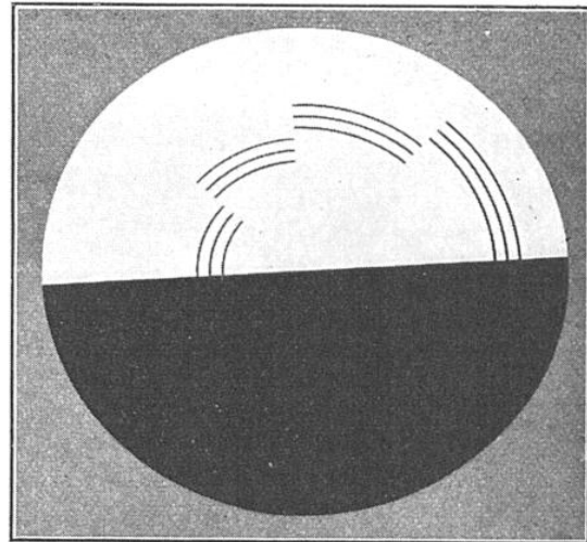
FIG. 2. — LE TOTON DE BENHAM
