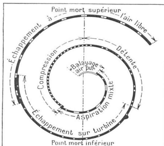
FIG. 4. — LES PHASES SUCCESSIVES DU CYCLE MOTEUR DANS UN DIESEL D'AVIATION A QUATRE TEMPS
