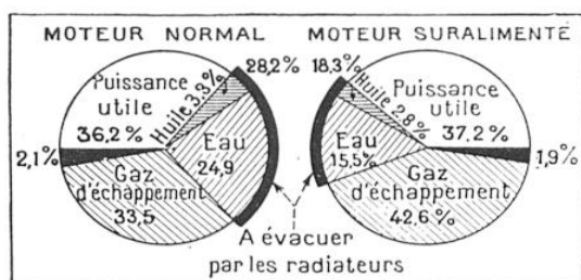
FIG. 5. — RÉPARTITION COMPARÉE DE L'ÉNERGIE CONSOMMÉE : A GAUCHE, DANS UN MOTEUR DIESEL NORMAL ; A DROITE, DANS UN DIESEL SURALIMENTÉ
