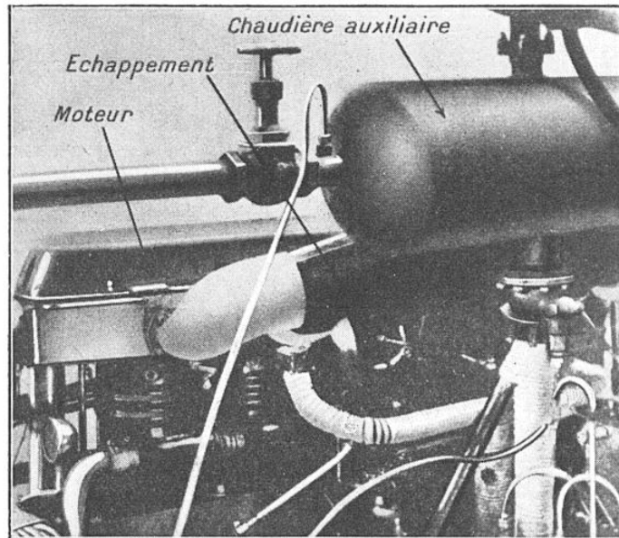
FIG. 3. — VOICI UN SYSTÈME NOUVELLEMENT ÉTUDIÉ PAR ISOTTA-FRASCINI SUR AVION « CAPRONI », EN VUE DE LA SURALIMENTATION EN ALTITUDE
