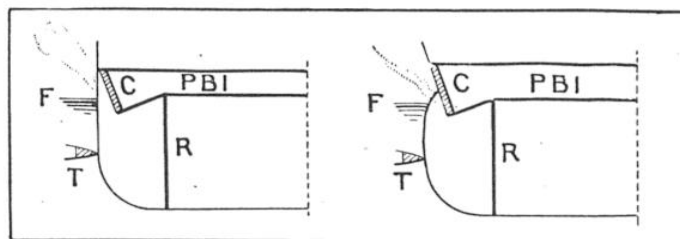
FIG. 10 ET 11. — COUPE AU MAITRE-COUPLE DE CUIRASSÉS A PROTECTION SOUS-MARINE MODERNE
