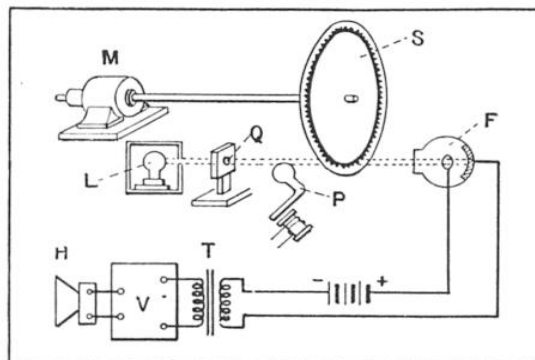
FIG. 1. — SCHÉMA DE PRINCIPE DE L'ORGUE PHOTOÉLECTRIQUE « WELTE »
