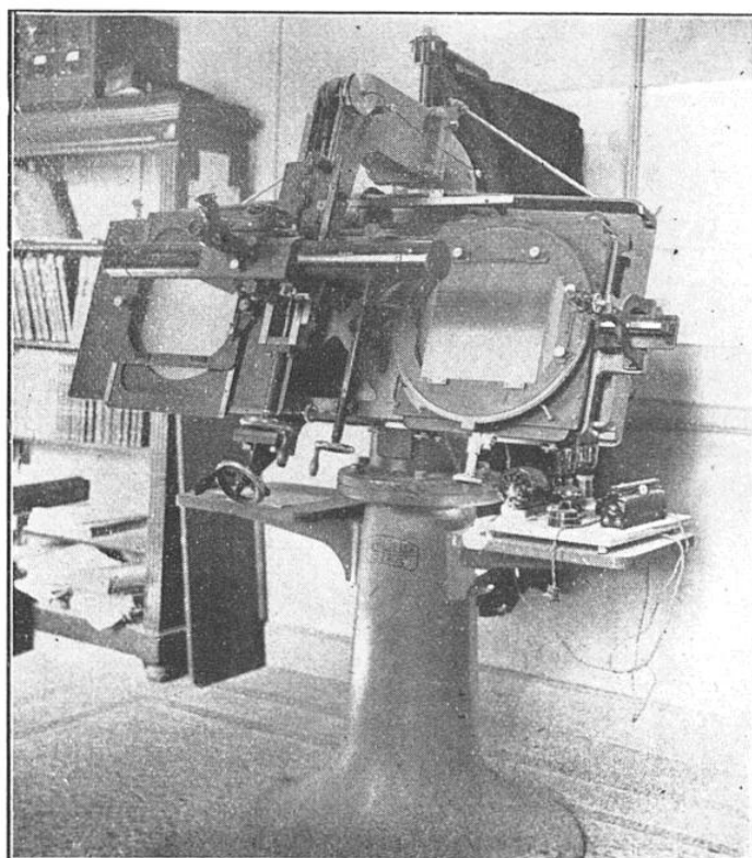
FIG. 4. — VUE D'ENSEMBLE DU « BLINK-MICROSCOPE »
