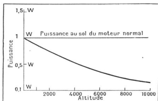
FIG. 1. — COURBE MONTRANT LA DÉGRESSION RAPIDE DE LA PUISSANCE W D'UN MOTEUR NORMAL EN FONCTION DE L'ALTITUDE
