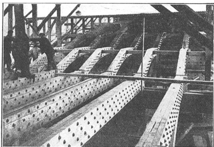
FIG. 1. — L'ASSEMBLAGE DE PLANCHES PERMET DE CONSTITUER DES POUTRES HOMOGÈNES A PARTIR D'UN MATÉRIAU HÉTÉROGÈNE : LE BOIS
