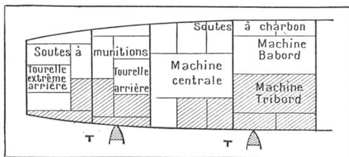
FIG. 1. — COUPE HORIZONTALE SCHÉMATIQUE SOUS LA FLOT- TAISON D'UN CUIRASSÉ ANCIEN A TROIS LIGNES D'ARBRES
