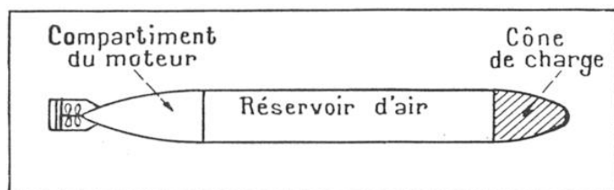
FIG. 7. — TORPILLE A PROPULSION PAR AIR COMPRIMÉ Les moteurs des torpilles récentes font plusieurs centaines de chevaux, et sont les plus légers de tous les types de moteurs (moins de 0,3 kg par ch). La charge d'explosif est voisine de 300 kg sur les derniers modèles. Le poids total atteint 1 800 kg sur les grandes torpilles « distance » de 533 à 550 mm de diamètre. Il est représenté, pour la plus grande partie, par le réservoir qui emmagasine l'air sous une pression de 250 à 300 kg/cm 2 .
