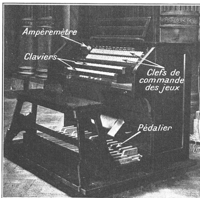
FIG. 3. — VUE D'ENSEMBLE DE LA CONSOLE DE L'ORGUE Cette console est en tout point analogue à celle d'un orgue pneumatique à commande électrique. Au-dessus des claviers, deux rangées de clefs permettent de faire entrer en action les différents jeux de l'orgue obtenus en modifiant le timbre des sons fondamentaux par l'adjonction d'harmoniques convenables.
