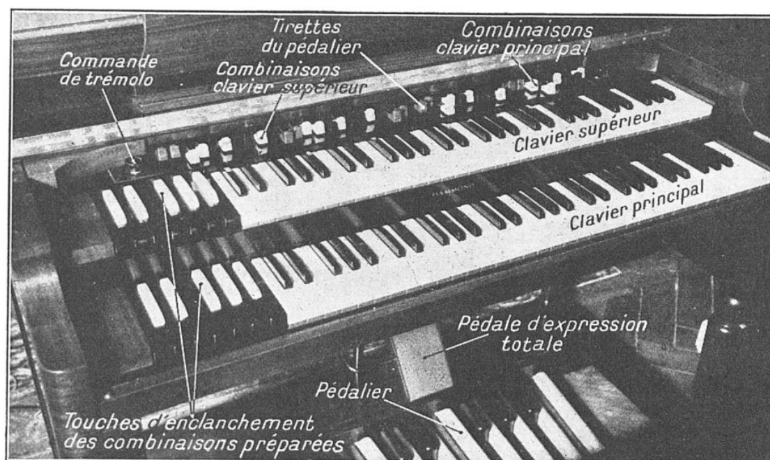
FIG. 7. — LES CLAVIERS DE L'ORGUE « HAMMOND »
