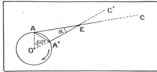
FIG. 7. — L'OBSERVATION DE LA PETITE PLANÈTE EROS PERMET DE MESURER LES DIMENSIONS DU SYSTÈME SOLAIRE
