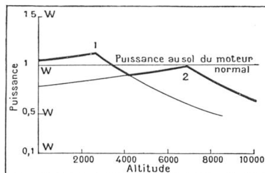
FIG. 2. — GRAPHIQUE MONTRANT LE « RÉTABLISSEMENT » DE LA PUISSANCE W EN ALTITUDE, PAR DEUX COMPRESSEURS ÉTAGÉS. La courbe 1 indique que la puissance unitaire d'un moteur comprimé dès le sol croît jusqu'à 2 400 m environ, pour décroître ensuite rapidement. Mais l'entrée en jeu du second étage de compression ramène un accroissement de puissance à partir de 4 000 jusqu'à 6 500 m environ, où la chute recommence. Il est évident qu'on ne peut « repêcher » la puissance par une succession indéfinie d'étages de compression qui absorbent eux-mêmes de la puissance motrice.
