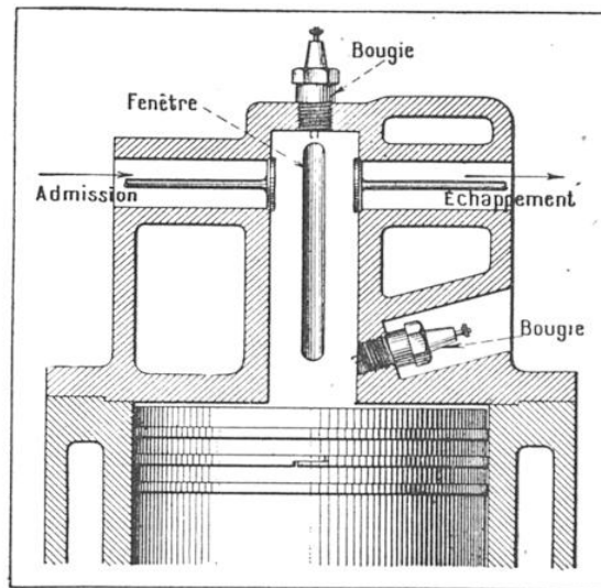
FIG. 6. — SCHÉMA DE LA CHAMBRE DE COMBUSTION DU MOTEUR A FENÊTRE UTILISÉ POUR L'ÉTUDE DE LA DÉTONATION
