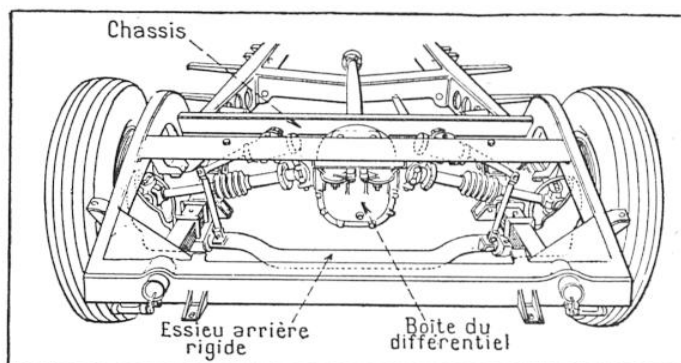
FIG. 8. — TRANSMISSION A DIFFÉRENTIEL SUSPENDU
