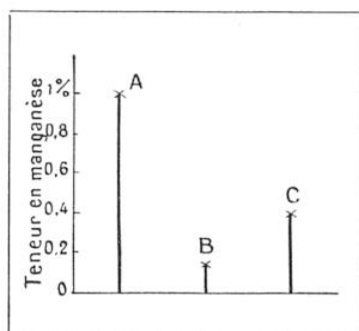
FIG. 1. — GRAPHIQUE MONTRANT LES TENEURS SUCCESSIVES EN MANGANÈSE AU COURS DE LA FABRICATION DE L'ACIER AU CONVERTISSEUR THOMAS
