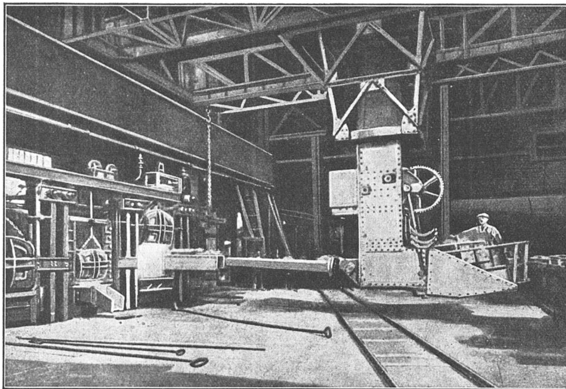
FIG. 3. — FOUR MARTIN FIXE DE 50 TONNES EN COURS DE CHARGEMENT
