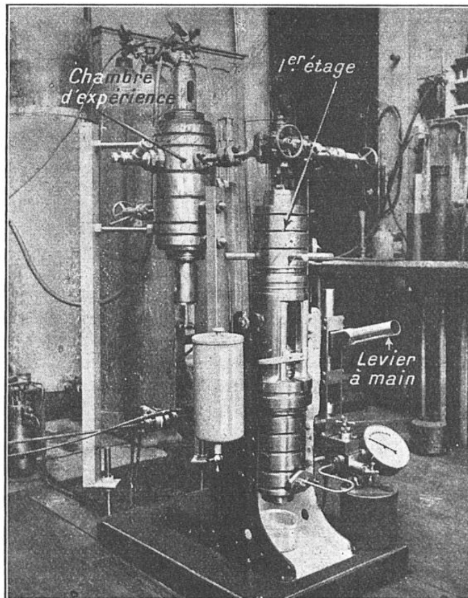
FIG. 1. — A L'AIDE DE CES PRESSES SPÉCIALES, M. JAMES BASSET RÉALISE DANS SON LABORATOIRE DES ULTRA-PRESSIONS DE L'ORDRE DE 40 000 KG/CM 2
