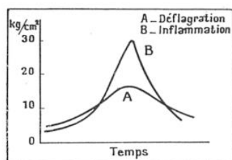
FIG. 10. — GRAPHIQUES TYPES DE LA COMBUSTION NORMALE ET DE LA DÉTONATION. La courbe A correspond à la déflagration normale ; la courbe B montre une augmentation brusque de la pression due au phénomène de détonation.
