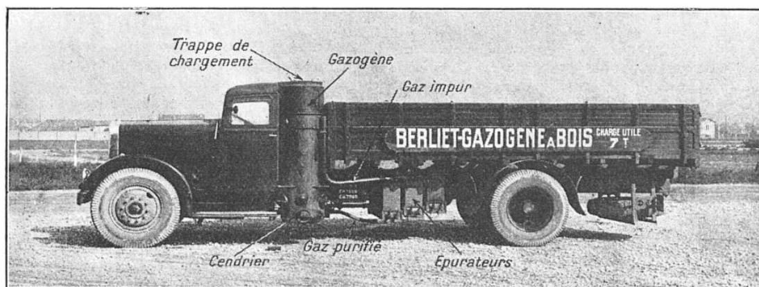
FIG. 11. — CAMION ALIMENTÉ PAR GAZOGÈNE AU BOIS
