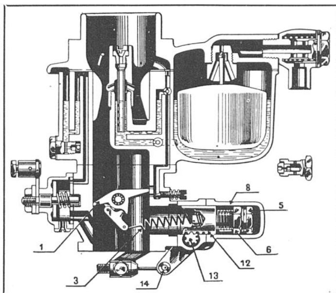
FIG. 2. — COUPE D'UN CARBURATEUR RÉGULATEUR « SOLEX » A VITESSE VARIABLE
