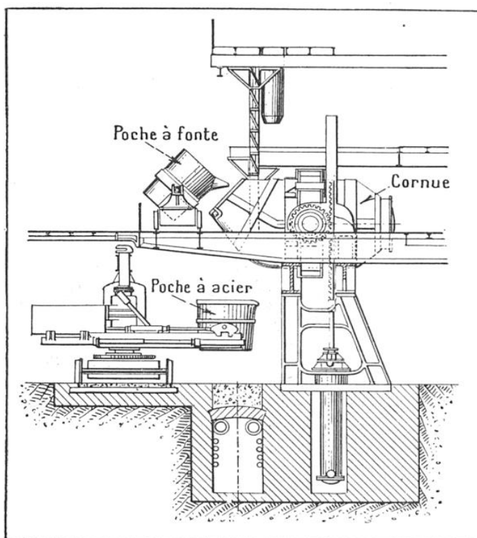
FIG. 2. — COUPE D'UNE ACIÉRIE THOMAS SIMPLE
