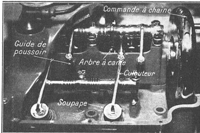
FIG. 2. — TÊTE D'UN MOTEUR 4 CYLINDRES EN V ET A CULBUTEURS POUR PETITE VOITURE
