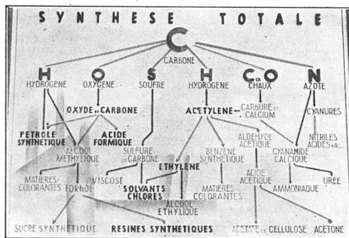
FIG. 1. — TABLEAU SCHÉMATIQUE DE LA SYNTHÈSE TOTALE DES PRODUITS ORGANIQUES À PARTIR DE L'ÉLÉMENT FONDAMENTAL : LE CARBONE
