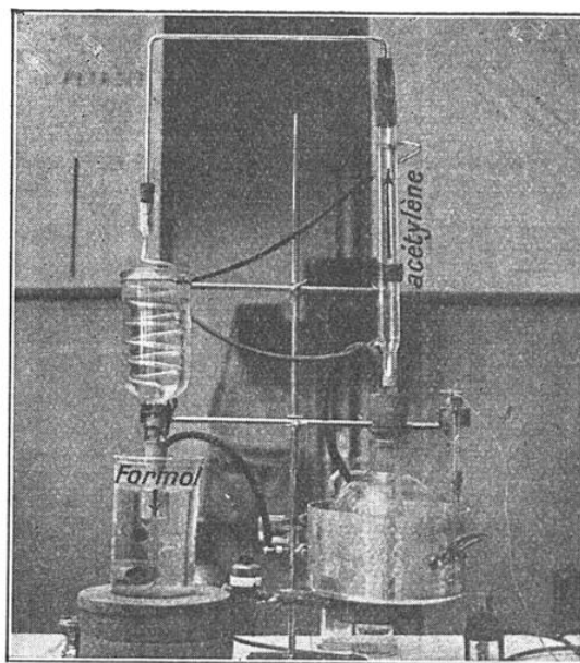
FIG. 3. — VOICI, A PARTIR DE L'ACÉTYLÈNE FABRIQUÉ CI-CONTRE, LA SYNTHÈSE DU FORMOL
