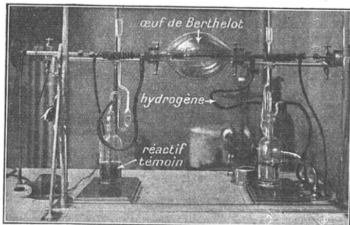
FIG. 2. — VOICI LA SYNTHÈSE DE L'ACÉTYLÈNE, TELLE QU'ELLE EST RÉALISÉE, D'APRÈS BERTHELOT, AU PALAIS DE LA DÉCOUVERTE (VOIR AUSSI PAGE CI-CONTRE)
