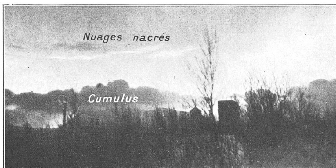
FIG. 1. — PHOTOGRAPHIE DE NUAGES NACRÉS OBSERVÉS EN SUÈDE SEPTENTRIONALE Ces nuages, de teintes rouges et vertes, observés à Abisko (Suède) par M. Chalonge, se distinguaient nettement des cumulus visibles à l'horizon. Ils étaient situés à l'altitude de 26 km environ.
