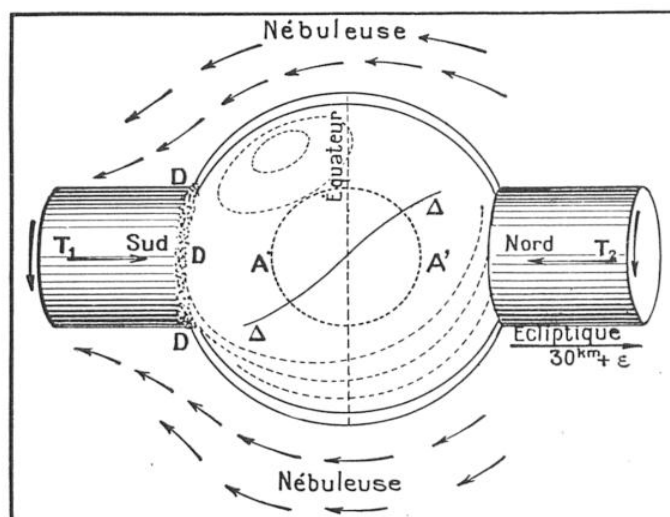
FIG. 2. — PAR SA CONDENSATION, LE TUBE-TOURBILLON INITIAL DONNE NAISSANCE AU SPHÉROÏDE TERRESTRE. Les deux extrémités T_1 et T_2 sont attirées l'une vers l'autre. Le premier noyau dense AA' entre à son tour en pulsation pour émettre cinq satellites dont quatre sont retombés plus tard sur la Terre. Le déluge austral primitif D donne naissance à toutes les mers. Le freinage qu'exerce la nébuleuse sur l'hémisphère nord provoque la déviation des continents austraux vers l'est, qu'indique la ligne \Delta .
