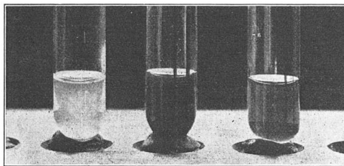
FIG. 3. - L'EFFET DES ULTRA-PRESSIONS SUR UNE DIASTASE
