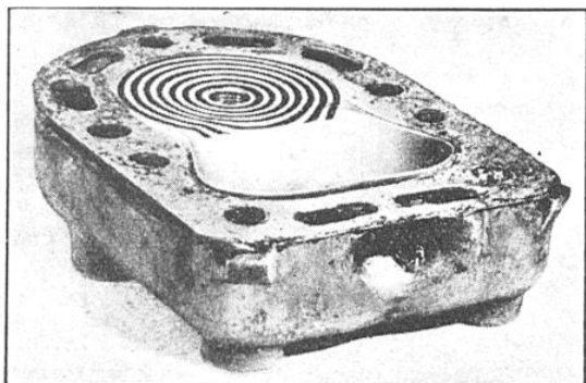
FIG. 12. — CULASSE STRIÉE EN ALPAX IMAGINÉE PAR M. SERRUYS POUR RETARDER L'APPARITION DE LA DÉTONATION
