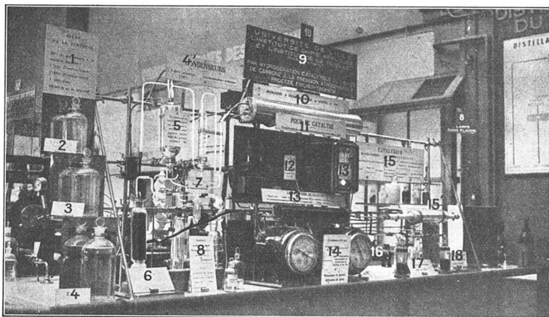
FIG. 5. — AU PALAIS DE LA DÉCOUVERTE FIGURE UN MODÈLE RÉDUIT DU DISPOSITIF COMPLEXE POUR LA SYNTHÈSE DE L'ESSENCE PAR LE PROCÉDÉ ALLEMAND FISCHER-TROPSCH
