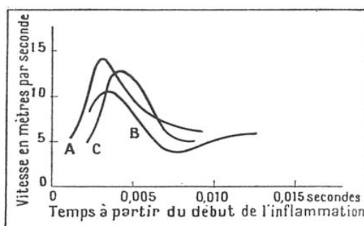
FIG. 1. — COMMENT SE PROPAGE LE « FRONT DE FLAMME » DANS LA COMBUSTION D'UN MÉLANGE GAZEUX EXPLOSIF
