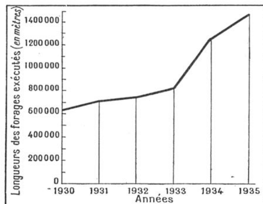
FIG. 4. — LA LONGUEUR DES FORAGES EXÉCUTÉS EN U. R. S. S. S'EST ACCRUE CONSIDÉRABLEMENT, MAIS DEMEURE CEPENDANT AU-DESSOUS DES CHIFFRES PRÉVUS DANS LES PLANS QUINQUENNAUX
