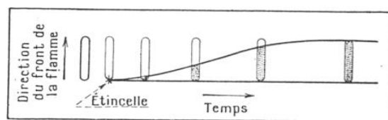
FIG. 7. — SCHÉMA MONTRANT COMMENT S'EFFECTUE L'ENREGISTREMENT DES PHÉNOMÈNES DE COMBUSTION ET DE DÉTONATION AU MOYEN DU MOTEUR A FENÊTRE (FIG. 6)
