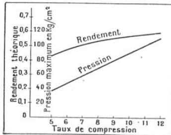
FIG. 5. — COMMENT VARIE LE RENDEMENT D'UN MOTEUR A EXPLOSIONS AVEC LE TAUX DE COMPRESSION
