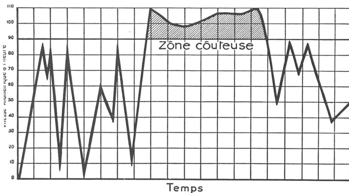
FIG. 1. — DIAGRAMME DE VITESSE MONTRANT QUE L'ON PEUT, EN AMÉLIORANT LA RÉGULARITÉ DE MARCHÉ, SUPPRIMER LES ZONES CÔUTEUSES ET CONSERVER LA MÊME MOYENNE (CARBURATEUR SOLEX)
