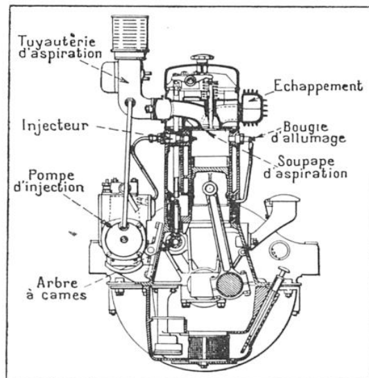
FIG. 6. — COUPE SCHÉMATIQUE D'UN MOTEUR D'AUTOMOBILE A INJECTION DE GAS OIL ET A ALLUMAGE PAR BOUGIE
