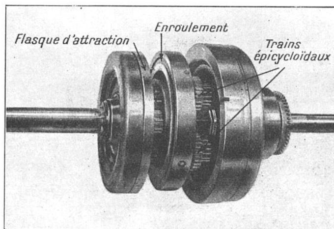
FIG. 3. — DÉTAIL DU MÉCANISME D'UN CHANGEMENT DE VITESSES ÉLECTROMAGNÉTIQUE
