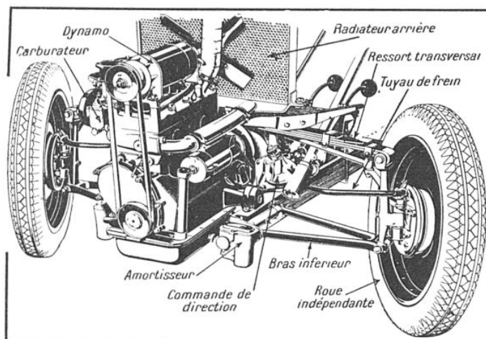
FIG. 1. — PARTIE AVANT DU CHASSIS DE LA « SIMCACINQ ». Remarquer l'extrême surbaisssement du moteur, sa position très avancée qui fait reporter le radiateur derrière lui, les roues avant indépendantes sur parallélogrammes déformables, dont un côté est constitué par le ressort transversal, l'autre par un triangle articulé commandant l'amortisseur hydraulique.
