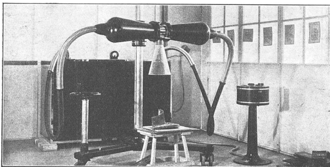
FIG. 1. — ENSEMBLE DU DISPOSITIF POUR LE CONTRÔLE RADIOGRAPHIQUE DES ORGANES MÉTALLIQUES DANS UN LABORATOIRE INDUSTRIEL MODERNE
