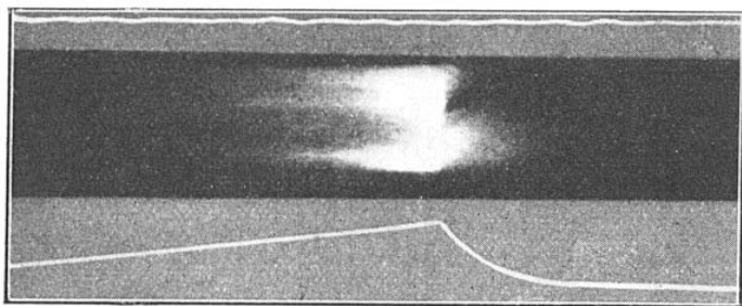
FIG. 8. — COMBUSTION DÉTONANTE ET DIAGRAMME DE LA PRESSION ENREGISTRÉS SIMULTANÉMENT AUX COURS D'ESSAIS EFFECTUÉS AVEC LE MOTEUR A FENÊTRE
