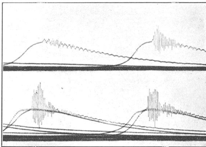
FIG. 9. — PORTIONS DE DIAGRAMMES OBTENUS AVEC LE MANOGRAPHE OPTIQUE DE M. SERRUYS
