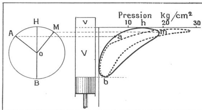
FIG. 4. — COMMENT EST RELEVÉ LE DIAGRAMME DE LA COMBUSTION DANS LE CYLINDRE D'UN MOTEUR A EXPLOSIONS H correspond au point mort haut et B au point mort bas ; v est le volume de la chambre d'explosion et V celui de la cylindrée. L'angle AOH est appelé avance à l'allumage, ce dernier s'effectuant en A. Le diagramme pression-volume tracé en trait plein correspond au régime normal du moteur ; celui en pointillé se rapporte au régime détonant.
