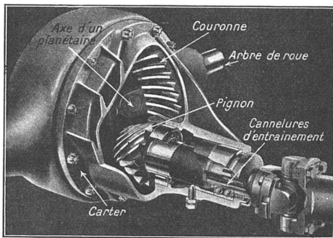
FIG. 10. — MÉCANISME DU PONT ARRIÈRE DIT « HYPOÏDE » Le pignon d'attaque, à denture de forme complexe, se trouve ici placé au-dessous de l'axe de la couronne. Le surbaissement de l'arbre de transmission qui en résulte avantage la position de carrosserie ; mais les effets de glissement (en plus du roulement relatif) qui prennent naissance entre les dentures provoquent parfois des érosions de celles-ci, si le graissage n'est pas confié à des lubrifiants spéciaux, du type Extrême-Pression .
