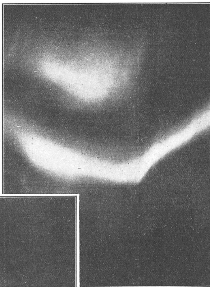
FIG. 3. — LA MÊME AURORE POLAIRE PHOTOGRAPHIÉE DANS SA PARTIE SUD SE PRÉSENTE SOUS UN ASPECT NETTEMENT DIFFÉRENT
