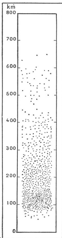
FIG. 6. — VOICI, D'APRÈS LES OBSERVATIONS DE STÖRMER, LES ALTITUDES OU ONT ÉTÉ OBSERVÉES LES AURORES POLAIRES, EN NORVÈGE MÉRIDIONALE, ENTRE 1911 ET 1922. C'est entre 100 et 200 km d'altitude que les aurores se rencontrent le plus fréquemment.
