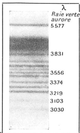
FIG. 7. — SPECTRE DU CIEL NOCTURNE OBTENU A VILLENES (SEINE-ET-OISE), EN FÉVRIER 1936, PAR M. ARNULF
