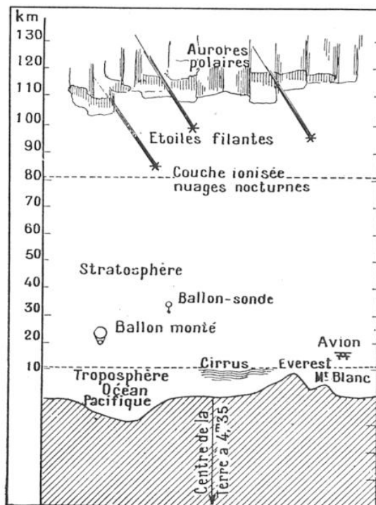
FIG. 4. — COUPE THÉORIQUE DE L'ATMOSPHÈRE JUSQU'À L'ALTITUDE DE 130 KM OU S'OBSERVENT LE PLUS GÉNÉRALEMENT LES AURORES POLAIRES
