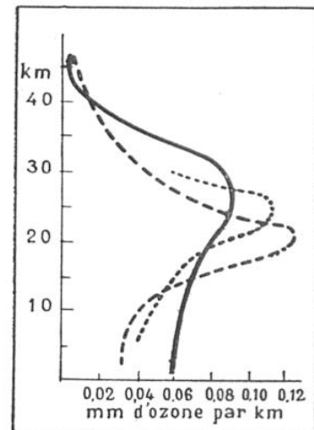
FIG. 5. — GRAPHIQUE MONTRANT LA DISTRIBUTION DE L'OZONE SUIVANT L'ALTITUDE. Les courbes en trait plein et en tirets sont dues à Götz, Meetham et Dolson ; celle en pointillé, à Regener.
