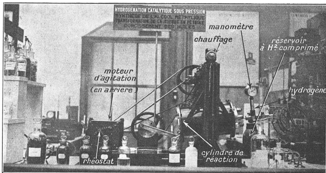
FIG. 4. — PAR HYDROGÉNATION CATALYTIQUE ET SOUS PRESSION DE L'OXYDE DE CARBONE, VOICI LA SYNTHÈSE DE L'ALCOOL MÉTHYLIQUE
