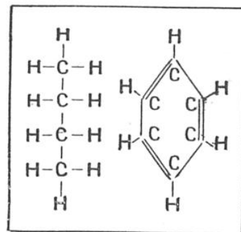
FIG. 13. — UN CARBURE A CHAÎNE OUVERTE ET UN CARBURE A CHAÎNE FERMÉE
