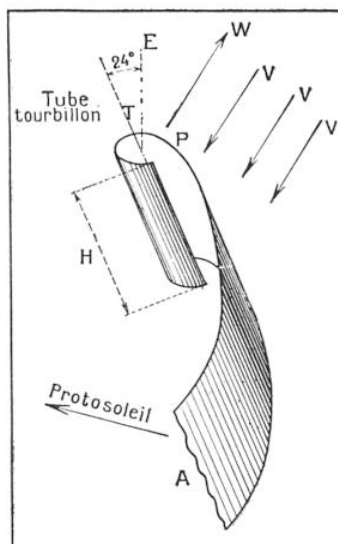
FIG. 1. — COMMENT S'EST FORMÉ LE TUBE-TOURBILLON QUI DONNA NAISSANCE À LA TERRE
