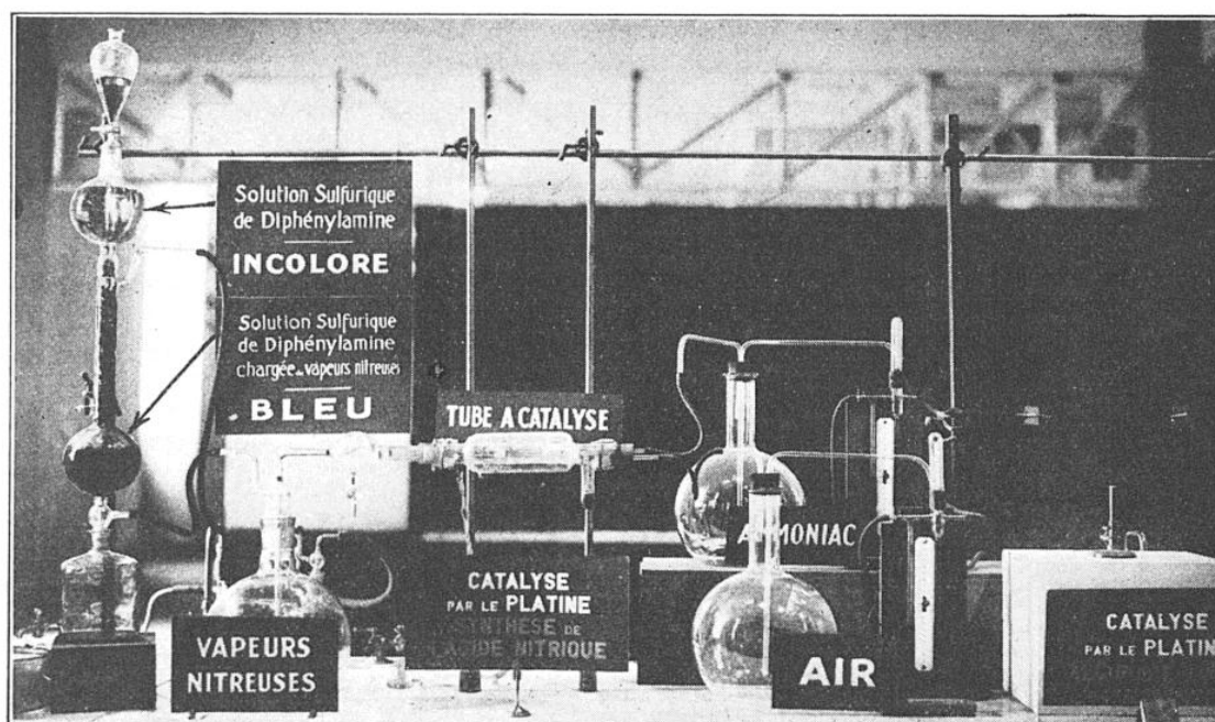
FIG. 6. — REPRÉSENTATION TRÈS SCHÉMATIQUE DE L'UNE DES SYNTHÈSES LES PLUS IMPORTANTES POUR L'INDUSTRIE : CELLE DE L'ACIDE NITRIQUE
