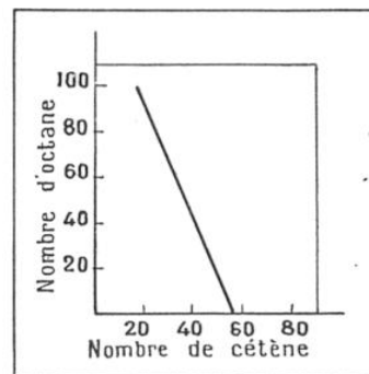
FIG. 11. — GRAPHIQUE METTANT EN ÉVIDENCE LA RELATION ÉTROITE ENTRE LES NOMBRES D'OCTANE ET DE CÉTÈNE
