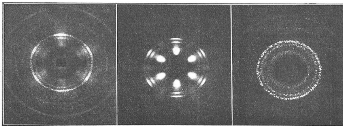
FIG. 2. — LA DIFFRACTION DES RAYONS X, QUI A FOURNI LES CLICHÉS CI-DESSUS, PERMET DE METTRE EN ÉVIDENCE LA « TEXTURE » DES MÉTAUX INDUSTRIELS ACQUISE AU COURS DE TRAITEMENTS MÉCANIQUES
