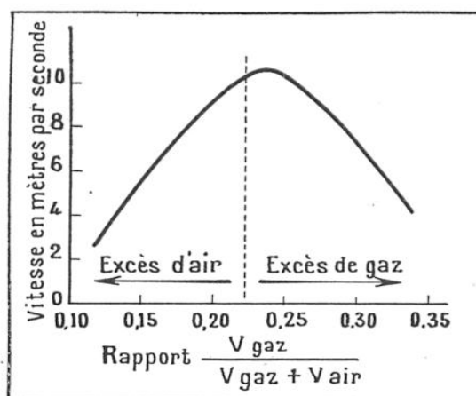
FIG. 2. — LA VITESSE DE COMBUSTION D'UN MÉLANGE EXPLOSIF VARIE D'UNE MANIÈRE CONSIDÉRABLE AVEC SA COMPOSITION
