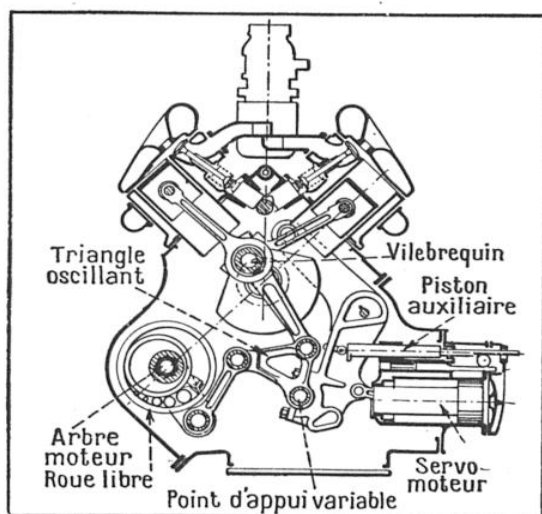
FIG. 7. — COUPE TRANSVERSALE DU MOTEUR ET DE LA TRANSMISSION AUTOMATIQUE R.V.R. Le triangle oscillant autour du point d'appui variable transforme le mouvement circulaire du vilebrequin, auquel il est lié, en impulsions alternatives qu'il communique à la roue libre. L'amplitude et la vitesse de ces impulsions varient avec la position du point fixe, qui est sous la dépendance du servo-moteur à action automatique, contrôlé par le piston auxiliaire, lié lui-même à l'accélérateur de la voiture.
