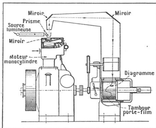
FIG. 3. — SCHÉMA DU MANOGRAPHE OPTIQUE A FAIBLE INERTIE DE M. SERRUYS
