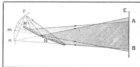
FIG. 6 ET 7. — DISPOSITIF EXPÉRIMENTAL POUR LA PRODUCTION DES FRANGES D'INTERFÉRENCE DE FRESNEL (A GAUCHE) ET SCHÉMA DE SON FONCTIONNEMENT (A DROITE)
