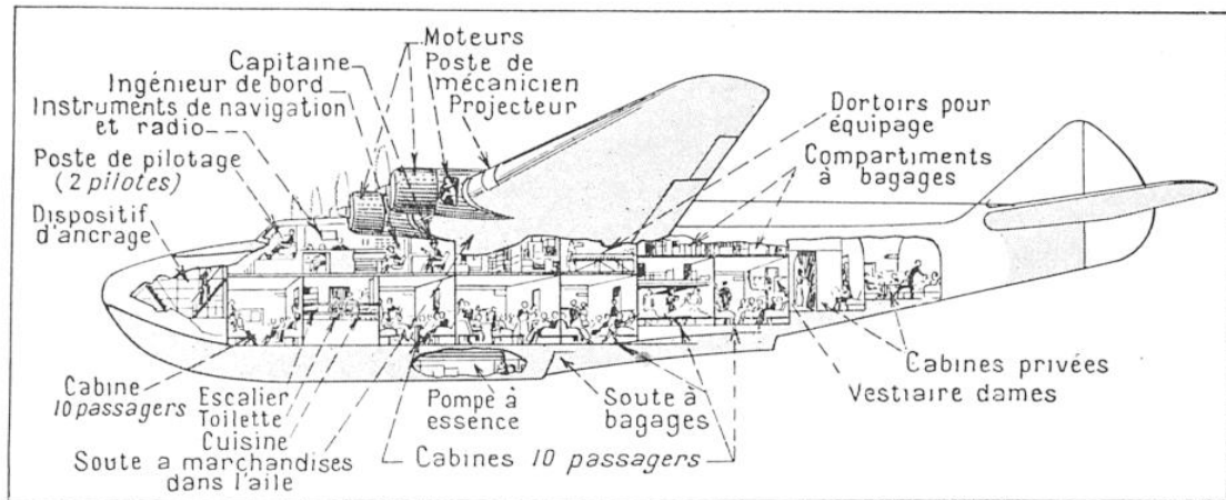
FIG. 7. — PLAN SCHÉMATIQUE DE L'AMÉNAGEMENT DE L'HYDRAVION TRANSATLANTIQUE AMÉRICAIN « BOEING-314 » DE 40 TONNES
