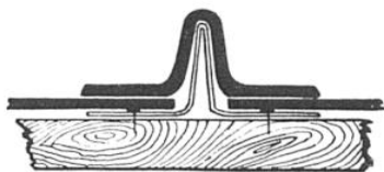
FIG. 2. — COUPE MONTRANT LA DISPOSITION DES BANDES DE « PAXALUMIN », DU SOUS-JOINT ET DU COUVRE-JOINT
