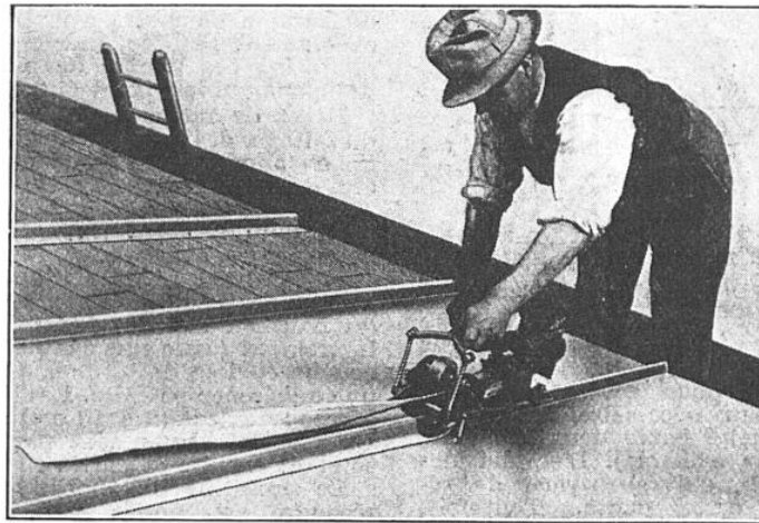
FIG. 1. — POSE A LA MACHINE D'UN COUVRE-JOINT « PAXALUMIN » SUR UNE TOITURE
