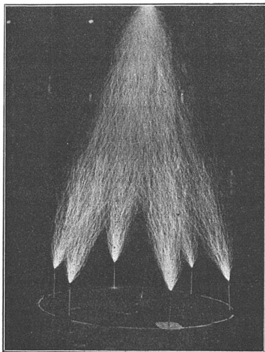
FIG. 7. — LES PARAFOUDRES A TIGES MULTIPLES ASSURENT UNE PROTECTION EFFICACE DE LA ZONE QU'ILS DÉLIMITENT
