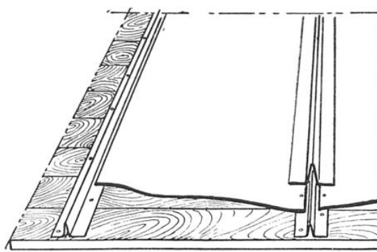
FIG. 3. — SCHÉMA D'UNE COUVERTURE EN « PAXALUMIN »
