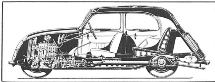
COUPE DE LA « SIMCA-8 »
