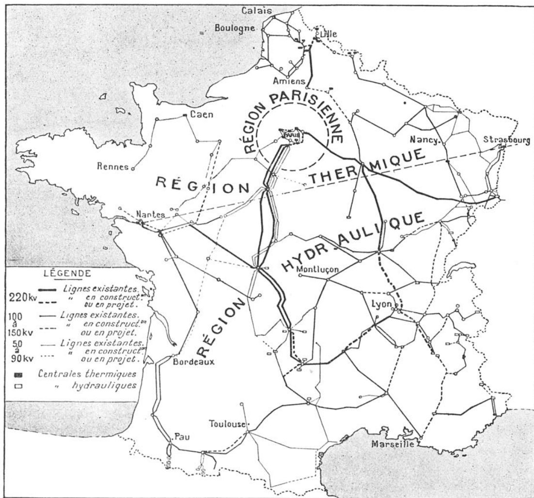
FIG. 1. — LE RÉSEAU FRANÇAIS D'INTERCONNEXION EN 1937
