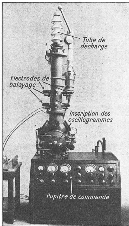
FIG. 4. — OSCILLOGRAPHE CATHODIQUE INSTALLÉ AU LABORATOIRE D'ÉTUDES DE M. ANGELINI, A TURIN (ITALIE)
