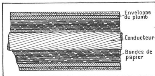
FIG. 2. — SECTION LONGITUDINALE D'UN CÂBLE A REMPLISSAGE GAZEUX
