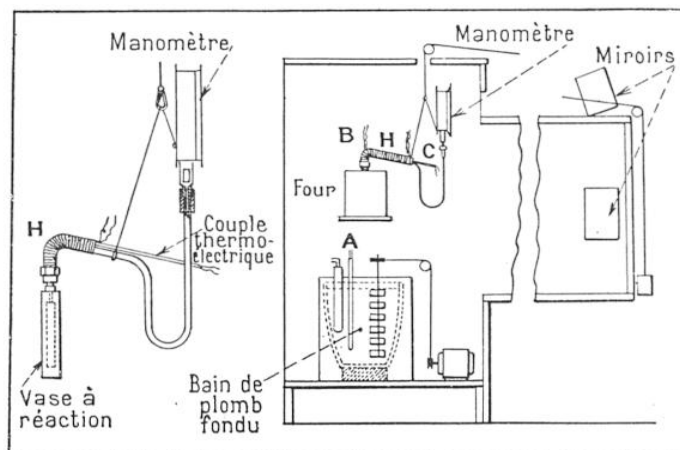
FIG. 4. — ENSEMBLE DE L'APPAREILLAGE POUR L'ÉTUDE DES VITESSES DE RÉACTION SOUS PRESSIONS ÉLEVÉES
