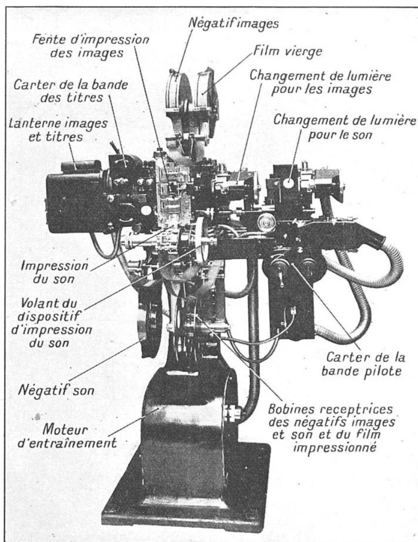
FIG. 4. — CETTE MACHINE A TIRER LES FILMS, LA PLUS MODERNE DU MONDE, EST CAPABLE D'IMPRESSIONNER 750 M DE FILM A L'HEURE. Cet appareil reporte sur un même film les images, le son et les sous-titres enregistrés séparément. Le film vierge et le négatif-images passent gélatine contre gélatine devant la fenêtre d'impression. Le négatif-images va alors s'enrouler sur sa bobine réceptrice, en bas. Le négatif-son est, à son tour, juxtaposé au film vierge, passe devant la fenêtre d'impression sonore, et les deux films s'enroulent sur leurs bobines réceptrices. La lumière fournie par la lanterne « images et titres » traverse la bande-titres, puis un jeu de lentilles, se réfléchit totalement sur un miroir en acier poli, puis traverse le négatif-images et le film vierge. La bande-pilote, enfermée dans le petit carter de droite, commande tous les mécanismes par l'intermédiaire de contacts électriques et de relais dont les fils sont protégés par des tubes métalliques flexibles.
