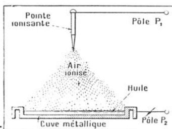
FIG. 1. — SCHÉMA DU DISPOSITIF PERMETTANT DE PRODUIRE AU LABORATOIRE LES TOURBILLONS CELLULAIRES THERMOCONVECTIFS ET ÉLECTROCONVECTIFS
