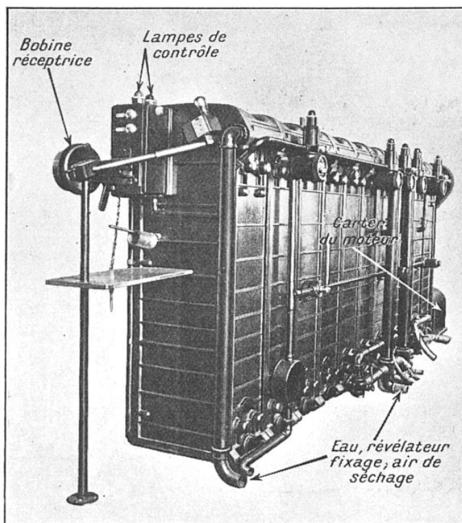
FIG. 3. — LA MACHINE CONTINUE A DÉVELOPPER LES FILMS CINÉMATOGRAPHIQUES « MULTIPLEX » VUE DE L'ARRIÈRE, COTÉ RÉCEPTEUR
