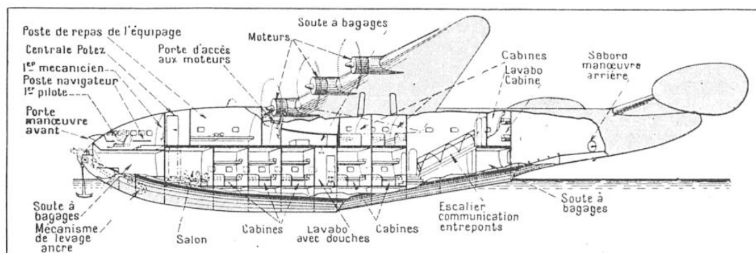
FIG. 10. — PLAN SCHÉMATIQUE D'AMÉNAGEMENT DE L'HYDRAVION TRANSATLANTIQUE DE 56 TONNES « LIORÉ-OLIVIER-49 » A SIX MOTEURS
