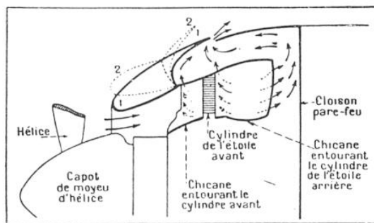
FIG. 4. — SCHÉMA DU REFROIDISSEMENT PAR L'AIR D'UN MOTEUR EN DOUBLE ÉTOILE, MONTRANT LES DEUX POSITIONS DES VOILETS MOBILES DU CAPOT
