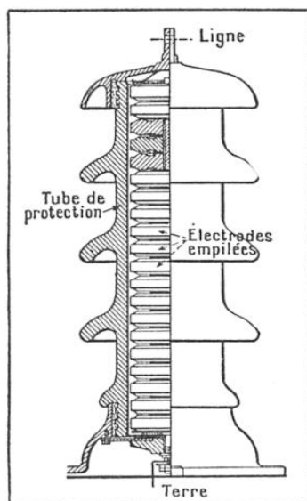
FIG. 5. — COUPE D'UN PARAFoudre LS A HAUTE TENSION
