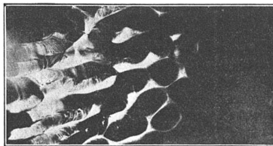
FIG. 13. — TOURBILLONS CELLULAIRES STATIONNAIRES RÉALISÉS AU LABORATOIRE
