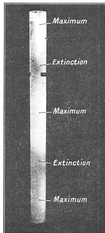
FIG. 26. — PHOTOGRAPHIE DU TUBE DE SOLUTION SUCRÉE OU SE MANIFESTE LA POLARISATION ROTATOIRE DE LA LUMIÈRE (EXPÉRIENCE DE LALLEMAND)
