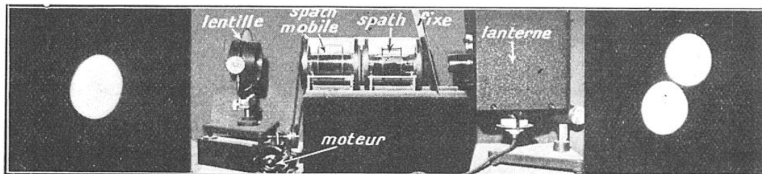
FIG. 16. — APPAREILLAGE POUR L'ÉTUDE DE LA BIRÉFRINGENCE DU SPATH
