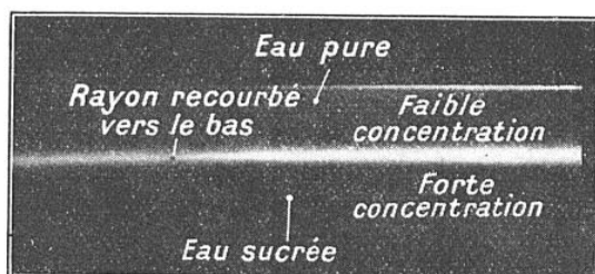
FIG. 2. — COURBURE D'UN RAYON LUMINEUX TRAVERSANT UNE SOLUTION SUCRÉE NON HOMOGÈNE (COURBURE VERS LE BAS)
