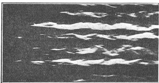
FIG. 7. — TOURBILLONS EN BANDES ALLONGÉES RÉALISÉS AU LABORATOIRE
