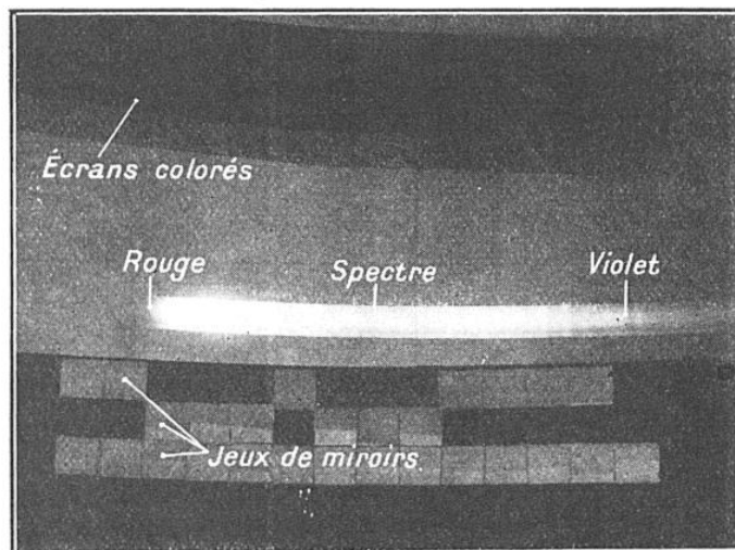
FIG. 5. — SPECTRE DE LA LUMIÈRE SOLAIRE PROJETÉ SUR LE MUR.
