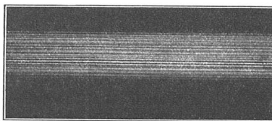
FIG. 8. — LES FRANGES D'INTERFÉRENCE DE FRESNEL PHOTOGRAPHIÉES SUR L'ÉCRAN E
