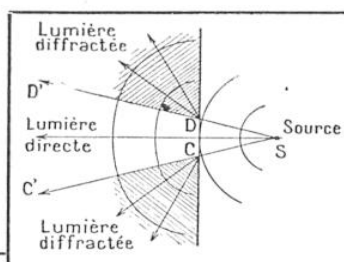
FIG. 11. — SCHÉMA DE PRINCIPE DE LA DIFFRACTION DE LA LUMIÈRE
