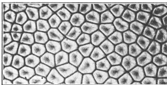
FIG. 2. — TOURBILLONS CELLULAIRES THERMOCONVECTIFS PHOTOGRAPHIÉS À LA SURFACE DE LA COUCHE D'HUILE (VOIR FIGURE 1)
