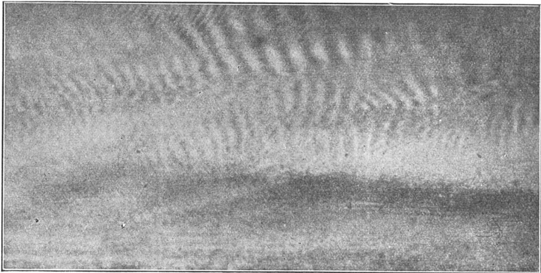
FIG. 9. — EXEMPLE DE NUAGES EN ROULEAUX TRANSVERSAUX
