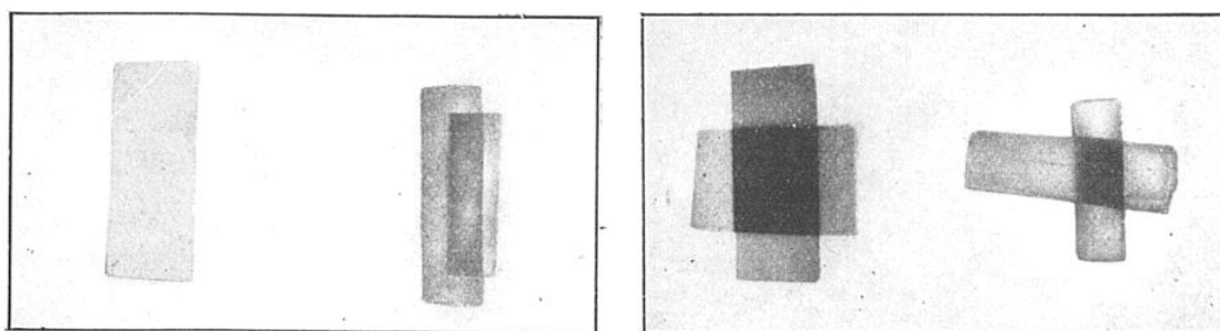
FIG. 18 ET 19. — LA POLARISATION PAR LES LAMES DE TOURMALINE ET D'HÉRAPATITE
