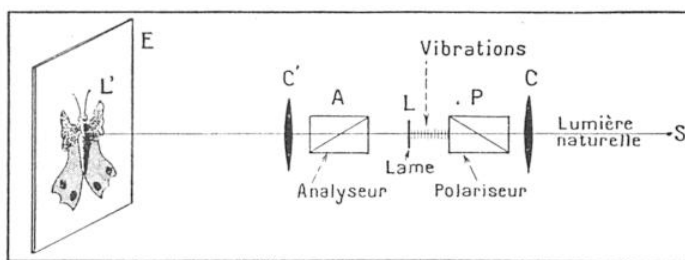
FIG. 20. — PRINCIPE DE LA POLARISATION CHROMATIQUE DES LAMES CRISTALLINES MINCES
