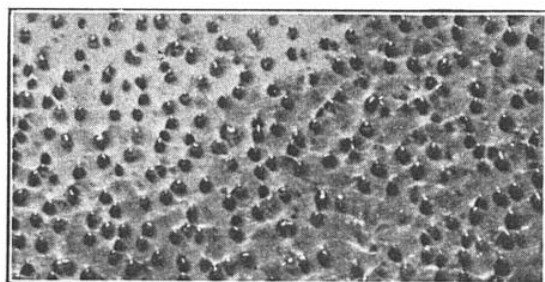
FIG. 3 ET 4. — TOURBILLONS CELLULAIRES ÉLECTROCONVECTIFS TELS QU'ON A PU LES PHOTOGRAPHIER AU LABORATOIRE ET LES OBSERVER À LA SURFACE DU SOLEIL
