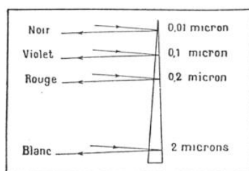
FIG. 9. — SCHÉMA DE PRINCIPLE MONTRANT LA COLORATION DES LAMES MINCES PAR INTERFÉRENCE
