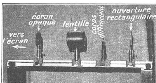
FIG. 12 ET 13. — COMMENT ON RÉALISE DES PROJECTIONS À L'AIDE DE LA LUMIÈRE DIFFRACTÉE
