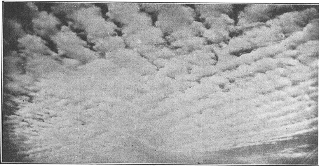
FIG. 12. — EXEMPLE DE NUAGES EN TOURBILLONS STATIONNAIRES
