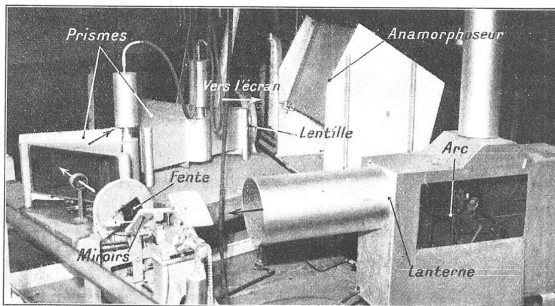
FIG. 4. — VUE D'ENSEMBLE DE LA PLATE-FORME RASSEMBLANT LES SOURCES DE LUMIÈRE ET L'APPAREILLAGE POUR L'ANALYSE SPECTRALE
