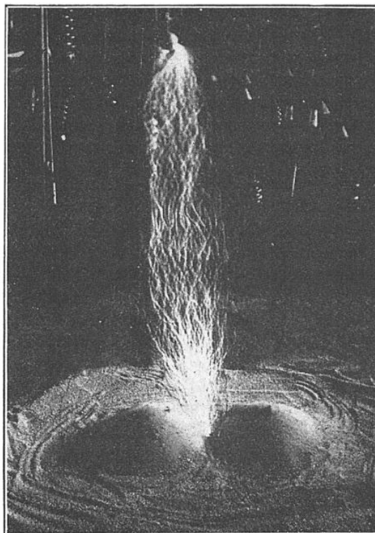
FIG. 8. — EXEMPLE DE FOUDROIEMENT « SÉLECTIF » OBTENU AU LABORATOIRE DE L'INSTITUT ÉLECTROTECHNIQUE DE L'U.R.S.S.
