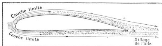
FIG. 5. — LES TOURBILLONS QUI SE FORMENT AU-DESSUS ET AU-DESSOUS DE L'AILE. A PARTIR DU POINT DU PROFIL DE L'AILE OU LA COUCHE LIMITE SE DÉSAGRÈGE, DONNENT NAISSANCE A UNE RÉSISTANCE CONSIDÉRABLE
