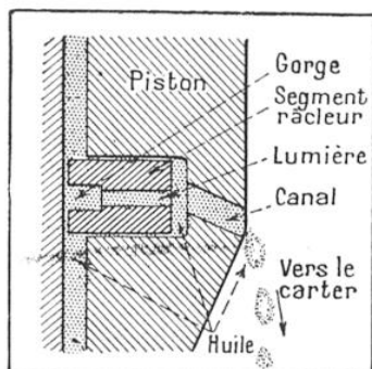
COUPE DU SEGMENT RACLEUR « REX » ASSURANT LE RETOUR DE L'HUILE AU CARTER
