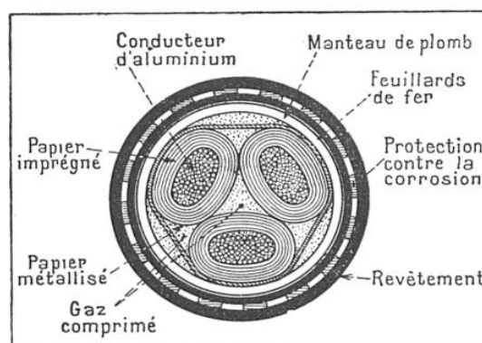
FIG. 3. — COUPE D'UN CÂBLE TRIPHASE A 33 000 VOLTS SOUS PRESSION DE GAZ
