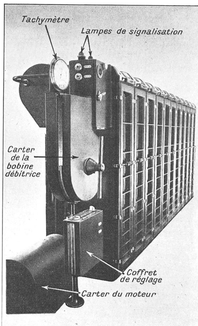
FIG. 2. — LA MACHINE CONTINUE A DÉVELOPPER LES FILMS CINÉMATOGRAPHIQUES « MULTIPLEX » VUE DE FACE. SON DÉBIT PEUT ATTEINDRE 2 100 M DE FILM A L'HEURE
