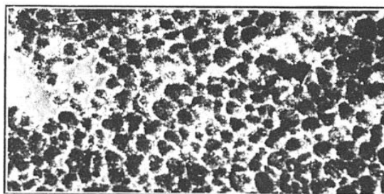
FIG. 3 ET 4. — TOURBILLONS CELLULAIRES ÉLECTROCONVECTIFS TELS QU'ON A PU LES PHOTOGRAPHIER AU LABORATOIRE ET LES OBSERVER À LA SURFACE DU SOLEIL
