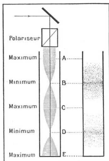
FIG. 25. — EXPÉRIENCES SUR LA POLARISATION ROTATOIRE D'UNE SOLUTION SUCRÉE
