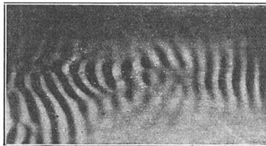
FIG. 10. — TOURBILLONS TRANSVERSAUX RÉALISÉS AU LABORATOIRE
