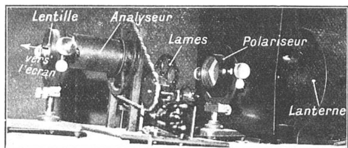
FIG. 21. — APPAREIL DE PROJECTION MONTRANT LA POLARISATION CHROMATIQUE PAR LES LAMES CRISTALLINES
