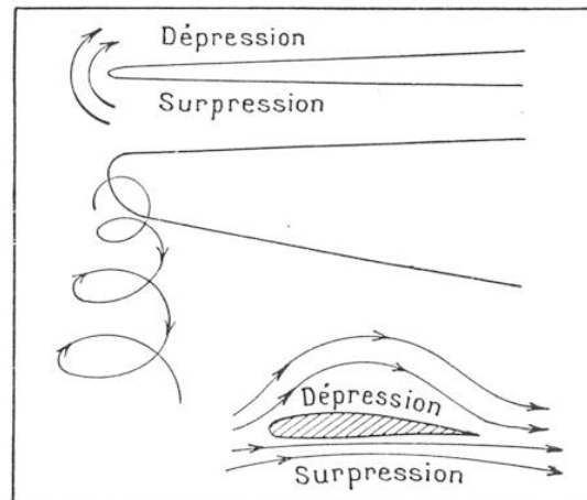
FIG. 6. — COMMENT PRENNENT NAISSANCE LES TOURBILLONS AUX EXTRÉMITÉS DES AILES. L'air comprimé par l'intrados tend à s'écouler vers l'extrados en contournant l'extrémité de l'aile. Il se forme donc un tourbillon quand l'avion se déplace.
