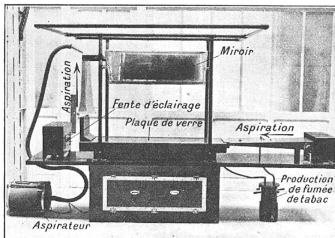
FIG. 5. — COMMENT ON RECONSTITUE EXPÉRIMENTALEMENT LES PHÉNOMÈNES THERMOCONVECTIFS DANS LES GAZ AU PALAIS DE LA DÉCOUVERTE
