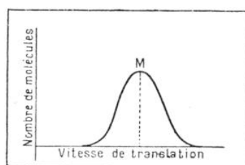
FIG. 1. — GRAPHIQUE MONTRANT LA RÉPARTITION DES VITESSES DE TRANSLATION ENTRE LES MOLÉCULES
