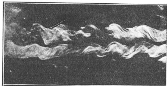
FIG. 8. — TOURBILLONS EN BANDES HÉLICOÏDALES RÉALISÉS AU LABORATOIRE
