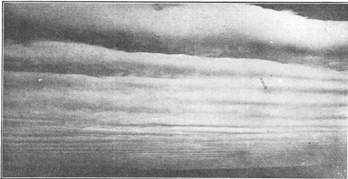
FIG. 6. — EXEMPLE DE NUAGES EN BANDES ALLONGÉES
