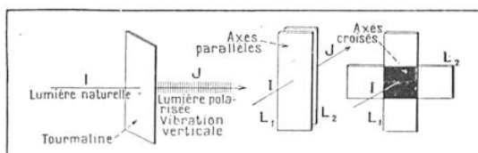
FIG. 17. — PRINCIPE DE LA POLARISATION DE LA LUMIÈRE PAR LA TOURMALINE
