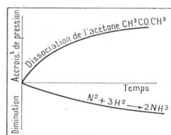
FIG. 2. — COMMENT VARIE LA PRESSION AU COURS D'UNE RÉACTION CHIMIQUE
