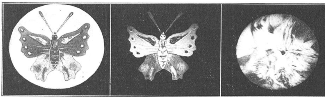
FIG. 22, 23 ET 24. — PROJECTIONS COLORÉES OBTENUES PAR LA POLARISATION CHROMATIQUE
