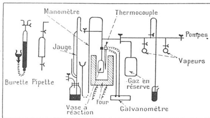
FIG. 3. — SCHÉMA D'UN APPAREIL DE LABORATOIRE POUR LA DÉTERMINATION DE LA VITESSE D'UNE RÉACTION CHIMIQUE PAR MESURE DE LA PRESSION
