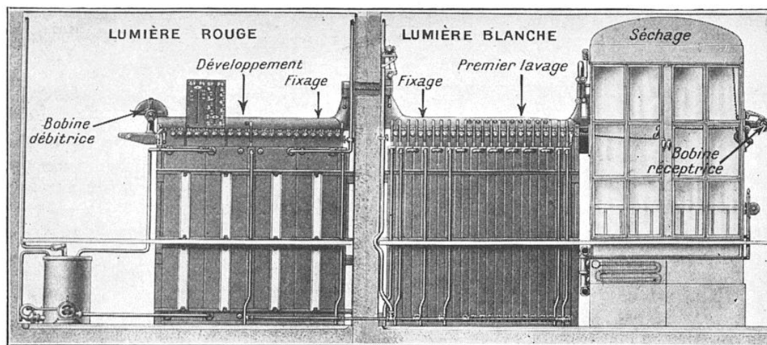
FIG. 1. — COUPE SCHÉMATIQUE D'UNE INSTALLATION POUR LE DÉVELOPPEMENT CONTINU ET TRÈS RAPIDE DES FILMS CINÉMATOGRAPHIQUES
