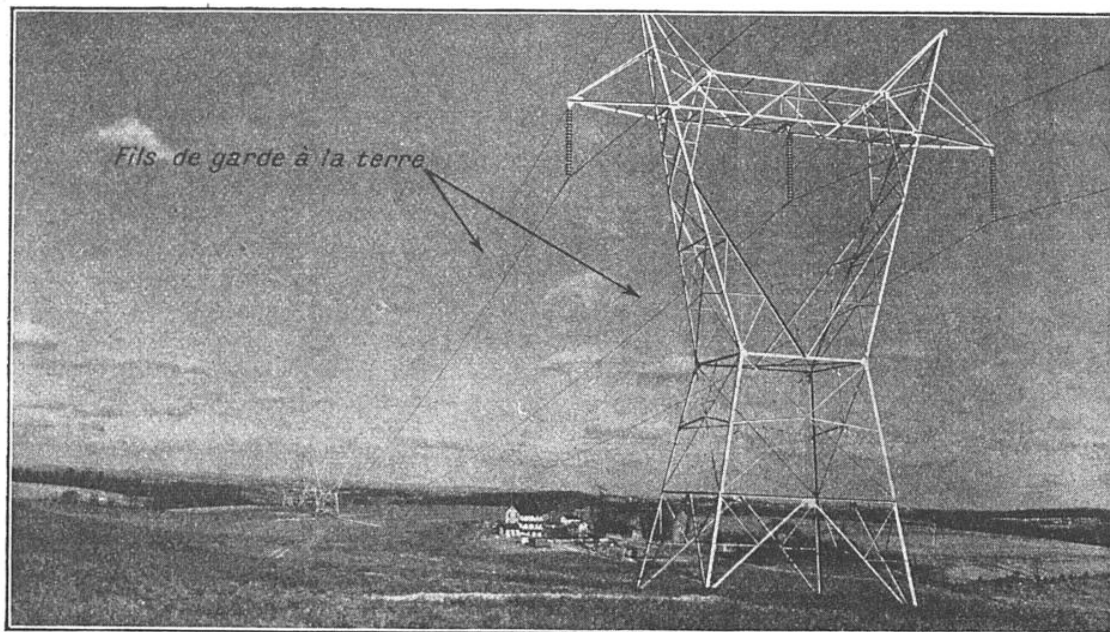
FIG. 9. — PYLONE DE SUSPENSION DE LA LIGNE AÉRIENNE A 230 000 VOLTS QUI RELIE LA CENTRALE DE SAFE HARBOUR AUX VILLES DE BALTIMORE ET WASHINGTON, AUX ÉTATS-UNIS. Cette ligne a une longueur de 147 km et sa protection contre la foudre a été spécialement étudiée. C'est ainsi que des fils de garde à la terre, placés très haut au-dessus des conducteurs, constituent un écran efficace pour la protection contre les coups de foudre directs. Les isolateurs de ligne sont formés par des chaînes de vingt éléments. Pour réduire la résistance de terre des pylônes, des contrepoids électriques (mises à la terre de grande surface judicieusement aménagées) ont été prévus. Depuis 1931, date de sa mise en service, cette ligne n'a subi qu'une seule interruption de deux minutes causée par la foudre.
