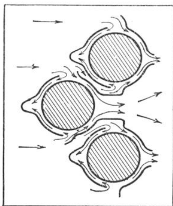
FIG. 3. — SCHÉMA DE LA CIRCULATION DE L'AIR AUTOUR DES CYLINDRES D'UN MOTEUR EN DOUBLE ÉTOILE
