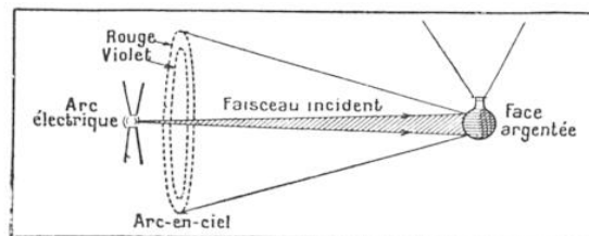
FIG. 1. — COMMENT EST PROJETÉ L'ARC-EN-CIEL SUR L'ENTRÉE DES SALLES D'OPTIQUE
