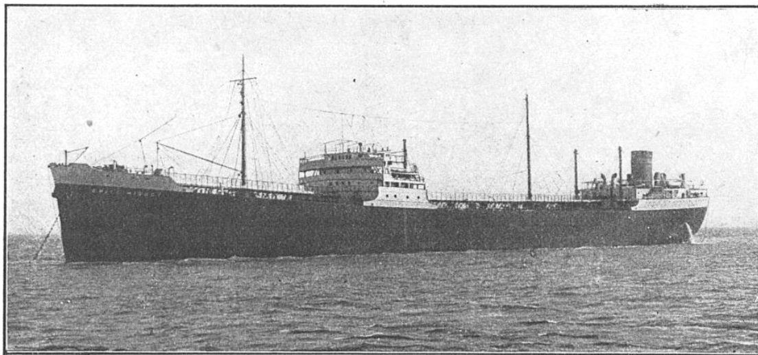
FIG. 5. — VOICI LE PLUS GRAND TANKER FRANÇAIS, L'« ÉMILE-MIGUET », DE 21 340 TONNES. Ce pétrolier, lancé en avril 1937, pour le compte de la Compagnie Navale des Pétroles, est destiné à importer en France les pétroles de l'Irak. Il est propulsé par deux moteurs Diesel de 6 cylindres, développant au total plus de 7 000 ch et lui donnant une vitesse de route de 13 nœuds.
