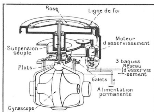
FIG. 2. — SCHÉMA DE FONCTIONNEMENT DU COMPAS GYROSCOPIQUE ASSERVI
