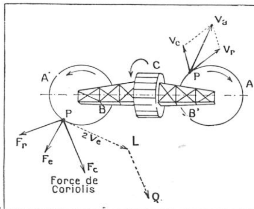
FIG. 8. — SCHÉMA DE LA RÉPARTITION DES VITESSES ET DES DIVERSES FORCES CENTRIFUGES DÉVELOPPÉES PAR LES ROTATIONS DANS LE « PERBALUM »
