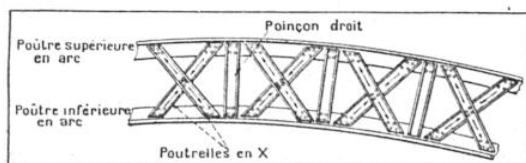
FIG. 3. — ARCHE FORMÉE DE POUTRES EN ACIER LAMINÉ ET RÉPARTITION DES EFFORTS DANS LE CROISILLONNAGE
