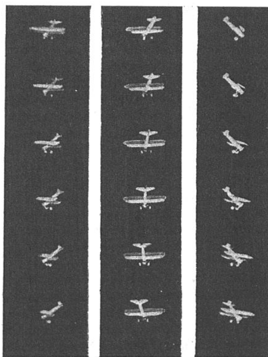
FIG. 5. — EXEMPLES DE FILMS CINÉMATOGRAPHIQUES DE « VRILLES » LIBRES RELEVÉS DANS LA SOUFFLERIE VERTICALE DU « N. A. C. A. », SPÉCIALISÉE DANS CETTE ÉTUDE
