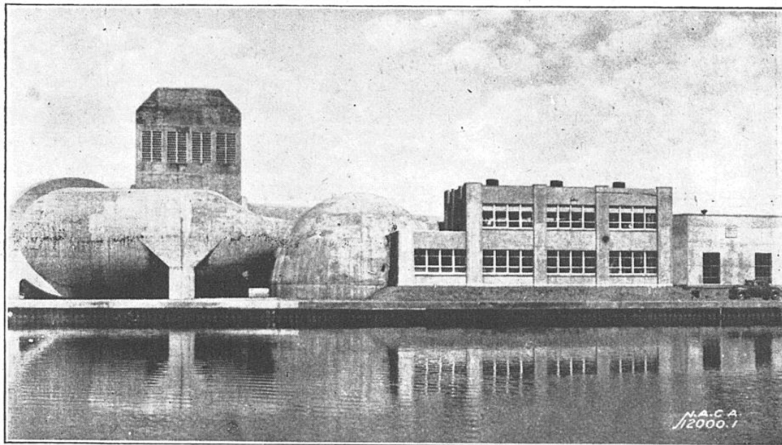
FIG. 3. — VUE GÉNÉRALE DE LA NOUVELLE SOUFFLERIE DU « N. A. C. A. » POUR LES ESSAIS A GRANDE VITESSE : LA VEINE FLUIDE A UN DIAMÈTRE UTILE DE 2 M 40 ET LA VITESSE DU COURANT D'AIR PEUT ATTEINDRE 850 KM/H
