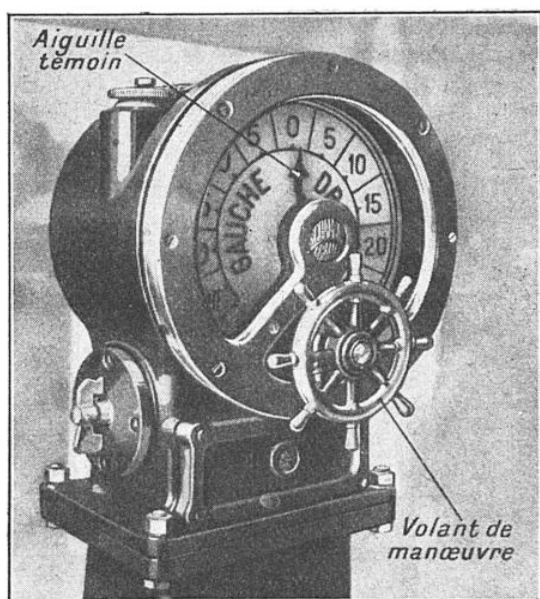
FIG. 4. — LE TRANSMETTEUR D'ORDRES DE LA PASSERELLE A LA BARRE
