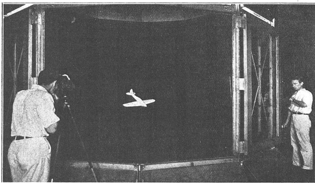
FIG. 4. — ÉTUDE CINÉMATOGRAPHIQUE DE LA « VRILLE » DANS LE TUNNEL VERTICAL SPÉCIAL DE 2 M DE DIAMÈTRE DU « N. A. C. A. », GRACE À UNE MAQUETTE D'AVION MAINTENUE PAR LE COURANT D'AIR À LA HAUTEUR DE LA CHAMBRE D'OBSERVATION.
