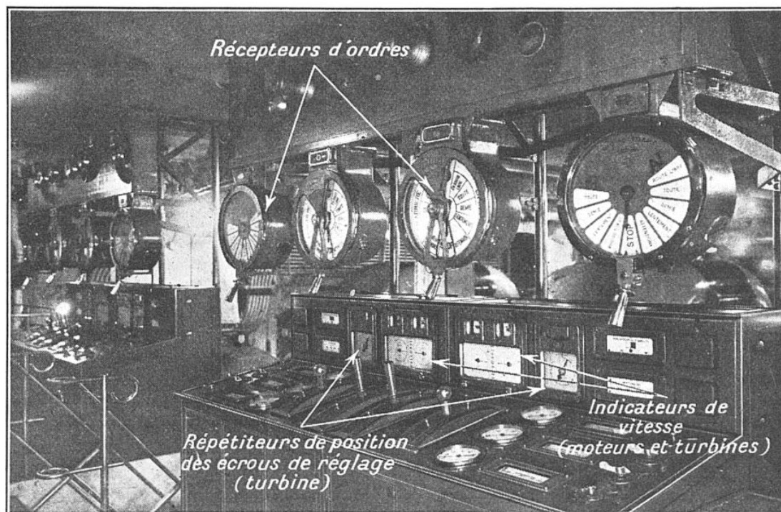
FIG. 7. — TABLEAU DE MANŒUVRE DE LA CHAMBRE DES MACHINES
