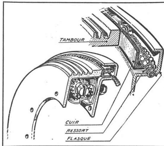
FIG. 10. — FREIN-ÉTANCHE « BENDIX » POUR VÉHICULES « TOUS TERRAINS »
