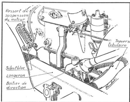
FIG. 4. — DÉTAILS DE LA SUSPENSION DU MOTEUR 402 « PEUGEOT »
