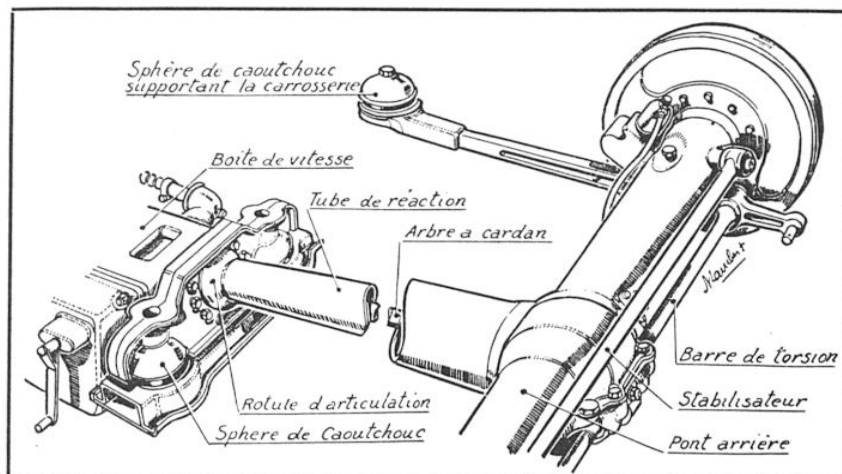
FIG. 8. — PONT ARRIÈRE DE LA NOUVELLE « PANHARD DYNAMIC »
