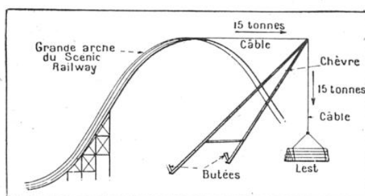
FIG. 5. — SCHÉMA DU DISPOSITIF UTILISÉ POUR LES ESSAIS DE SÉCURITÉ DE LA GRANDE ARCHE DU « SCENIC RAILWAY »
