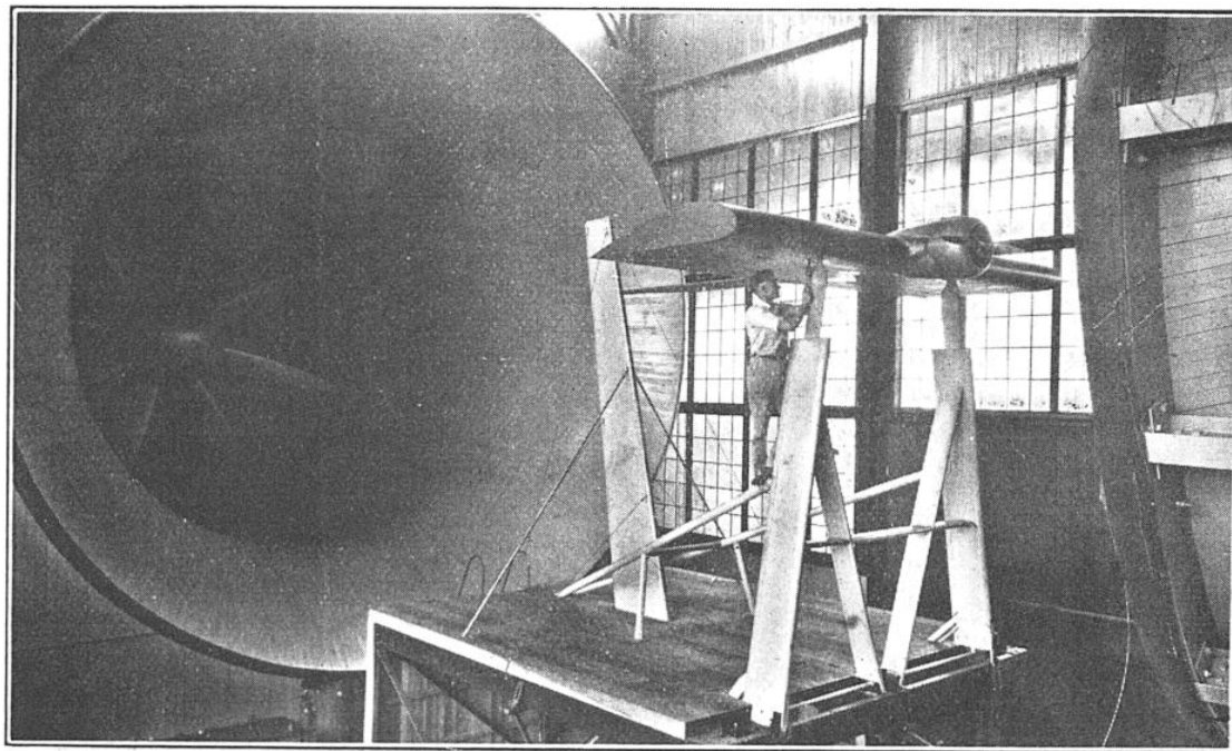
FIG. 2. — ÉTUDE DES INTERACTIONS ENTRE UNE AILE ET UNE HÉLICE ET DU CAPOTAGE D'UN MOTEUR DANS LA GRANDE SOUFFLERIE DE 6 M DE DIAMÈTRE DU « N. A. C. A. » A LANGLEY FIELD
