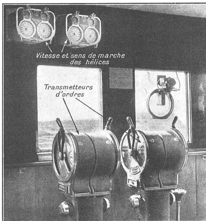
FIG. 6. — VOICI UN DES GROUPES DE TRANSMETTEURS-RÉPÉTEURS D'ORDRES AUX MACHINES INSTALLÉS SUR LA PASSERELLE DE LA « NORMANDIE »
