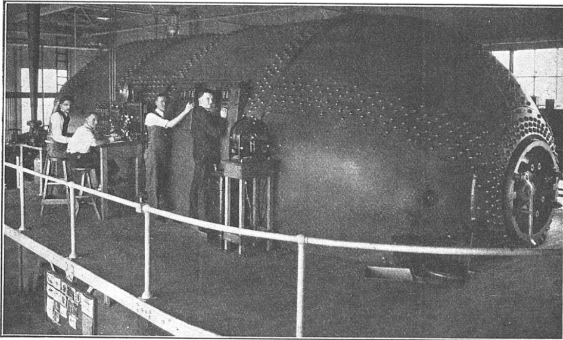
FIG. 1. — LA SOUFFLERIE SOUS PRESSION VARIABLE DU « N. A. C. A. » OU S'EFFECTUE L'ÉTUDE SYSTÉMATIQUE DES PROFILS D'AILES DANS DES CONDITIONS VOISINES DU VOL RÉEL
