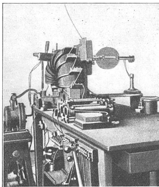
FIG. 6. — SPECTROGRAPHE DE MASSE DE F.-W. ASTON AU LABORATOIRE CAVENDISH, PERMETTANT DE DÉTERMINER LES MASSES ATOMIQUES AVEC UNE PRÉCISION ATTEIGNANT LE VINGT-MILLIÈME ET MÊME, PARFOIS, LE CENT-MILLIÈME
