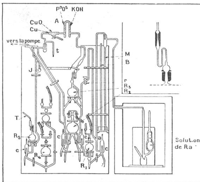
FIG. 3. — SCHÉMA DE L'APPAREIL SERVANT À L'EXTRACTION DE L'ÉMANATION DU RADIUM OU RADON
