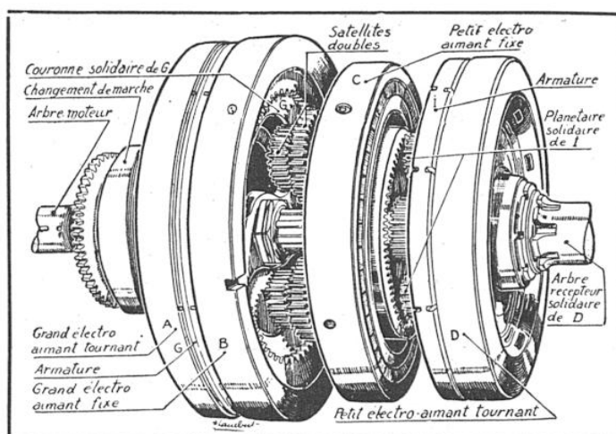
FIG. 6. - BOITE DE VITESSES ÉLECTROMAGNÉTIQUE « COTAL »
