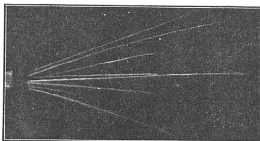
FIG. 9. — GERBE DE RAYONS H NATURELS (PROTONS) PRODUITS PAR LE PASSAGE DE RAYONS ALPHA DANS LA CELLOPHANE
