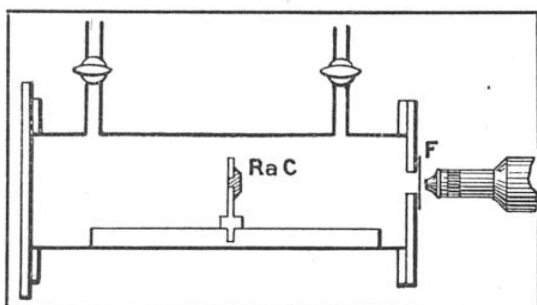
FIG. 7. — APPAREIL DE RUTHERFORD POUR LA DÉSINTÉGRATION DES ATOMES
