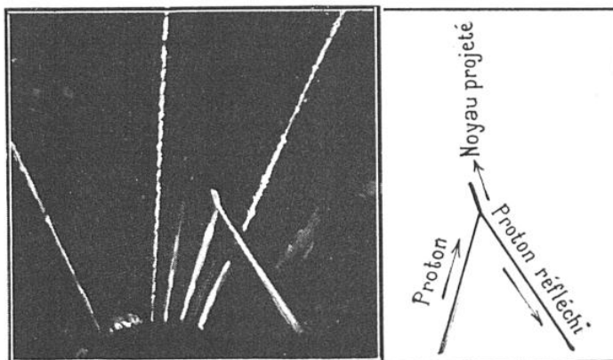
FIG. 11. — PHOTOGRAPHIE DE LA RENCONTRE D'UN RAYON H (PROTON) AVEC UN NOYAU D'OXYGÈNE
