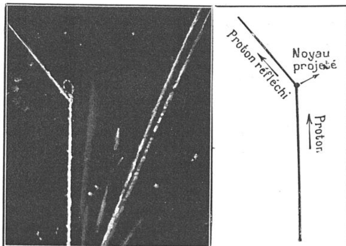
FIG. 10. — PHOTOGRAPHIE DE LA RENCONTRE D'UN RAYON H (PROTON) AVEC UN ATOME D'AZOTE
