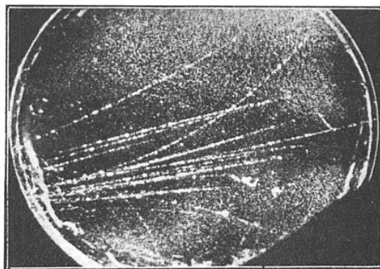
FIG. 13. — PHOTOGRAPHIE OBTENUE A LA CHAMBRE HUMIDE DE C.-T.-R. WILSON MONTRANT LA PRODUCTION D'ÉLECTRONS NÉGATIFS ET POSITIFS
