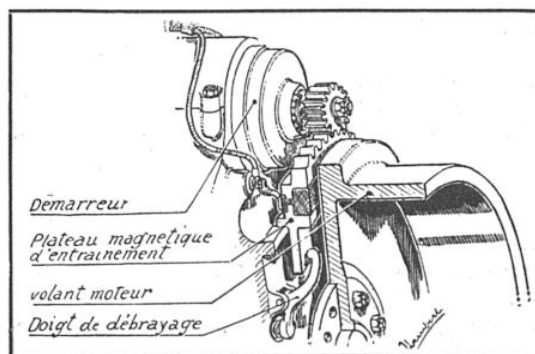
FIG. 7. — DÉMARREUR A PLATEAU MAGNÉTIQUE « PARIS-RHÔNE »
