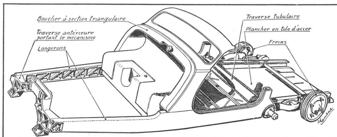
FIG. 2. — CHASSIS-CARCASSE « AMILCAR » CONSTITUANT A LA FOIS LE SUPPORT DES ORGANES MÉCANIQUES ET L'AMORCE DE LA CARROSSERIE
