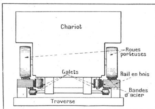
FIG. 4. — DISPOSITION DES GALETS DE SÉCURITÉ FORMANT ACCROCHAGE COMPLET DES CHARIOTS DU « SCENIC » A LA VOIE
