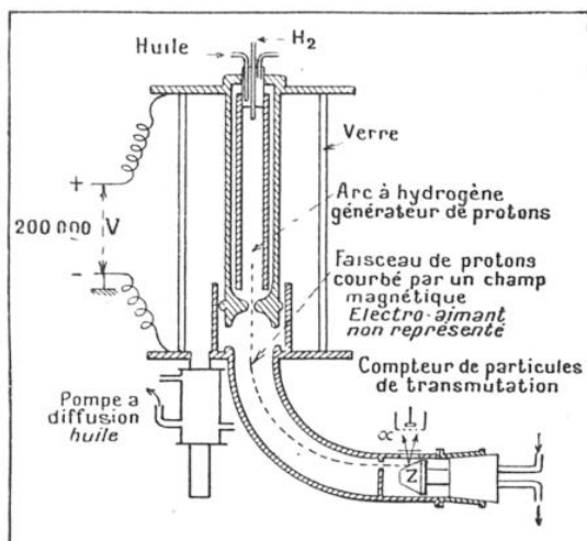
FIG. 8. — APPAREIL D'OLIPHANT ET RUTHERFORD POUR PRODUIRE LES TRANSMUTATIONS ATOMIQUES A L'AIDE D'UN FAISCEAU INTENSE DE PROTONS (NOYAUX D'HYDROGÈNE)
