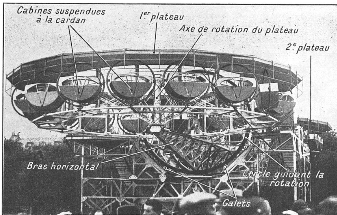
FIG. 7. — VUE D'ENSEMBLE DU « PERBALUM », APPAREIL A ROTATIONS COMPOSÉES
