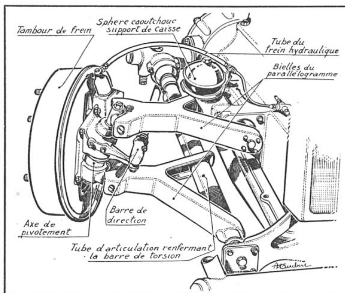
FIG. 3. — DÉTAIL DE LA SUSPENSION AVANT DE LA « PANHARD DYNAMIC »
