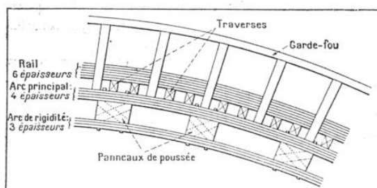
FIG. 2. — DÉTAIL DE LA CONSTRUCTION DES ARCHES EN BOIS, FORMÉES DE PLANCHES SUPERPOSÉES DE PIN ROUGE D'ORÉGON. Les croisillons pointillés sont fictifs : ils indiquent la correspondance avec les croisillons en acier d'une arche métallique (figure 3).
