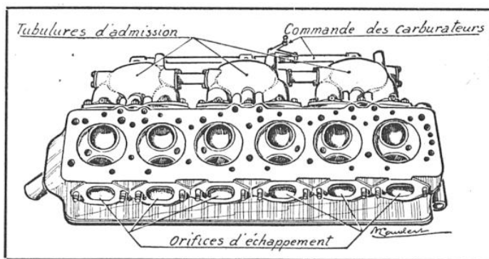
FIG. 5. - CULASSE EN ALPAX DU NOUVEAU MOTEUR « TALBOT »
