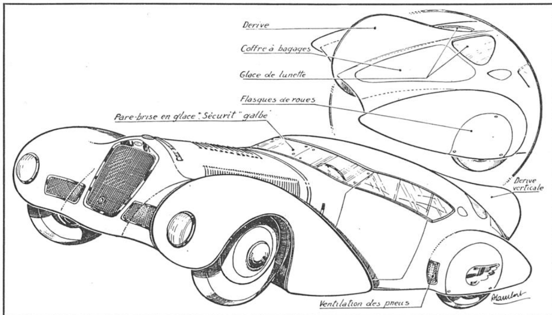
FIG. 1. - VOITURE « DELAGE » AVEC CARROSSERIE AÉRODYNAMIQUE « ANDREAU-LABOURDETTE » Cette voiture ne présente aucune saillie extérieure. Elle est munie à l'arrière d'une dérive dont le rôle est de rapprocher le centre de poussée du centre de gravité. Sa résistance à l'avancement dans l'air est au moins trois fois plus faible que celle d'une voiture normale. Le pare-brise, en glace « Sécurité » très épaisse, est utilisé comme élément de construction pour soutenir le pavillon.
