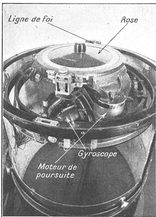
FIG. 1. — LE GYRO-COMPAS « SPERRY » AVEC ASSERVISSEMENT « SAINT-CHAMOND GRANAT »
