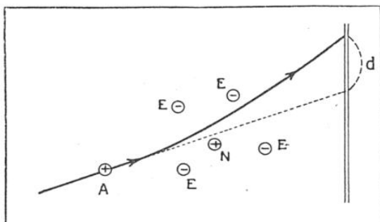
FIG. 5. — EXPÉRIENCE IMAGINÉE PAR RUTHERFORD ET PERMETTANT DE CALCULER LA CHARGE ÉLECTRIQUE POSITIVE DU NOYAU ATOMIQUE N PAR LA MESURE DE LA DÉVIATION d IMPRIMÉE À UN CORPUSCULE ALPHA A
