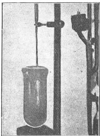
FIG. 2. — TUBE DE VERRE CONTENANT DU RADON (ÉMANATION DU RADIUM) CONDENSÉ À BASSE TEMPÉRATURE,
