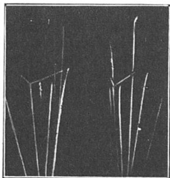
FIG. 12. — PHOTOGRAPHIE STÉRÉOSCOPIQUE OBTENUE DANS LA CHAMBRE HUMIDE DE C.-T.-R. WILSON MONTRANT LE CHOC D'UNE PARTICULE ALPHA CONTRE UN NOYAU D'OXYGÈNE
