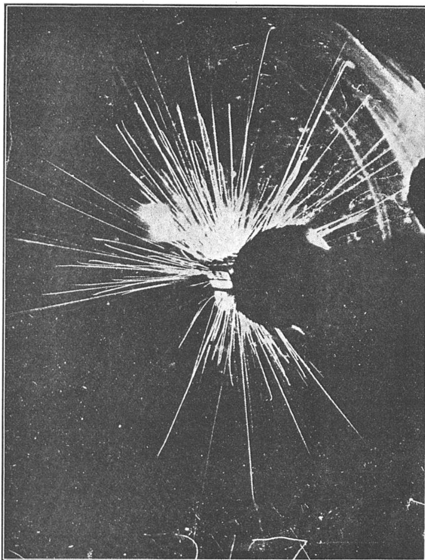
FIG. 4. — PHOTOGRAPHIE OBTENUE A LA CHAMBRE HUMIDE DE C.-T.-R. WILSON, MONTRANT LA TRANSMUTATION DU LITHIUM
