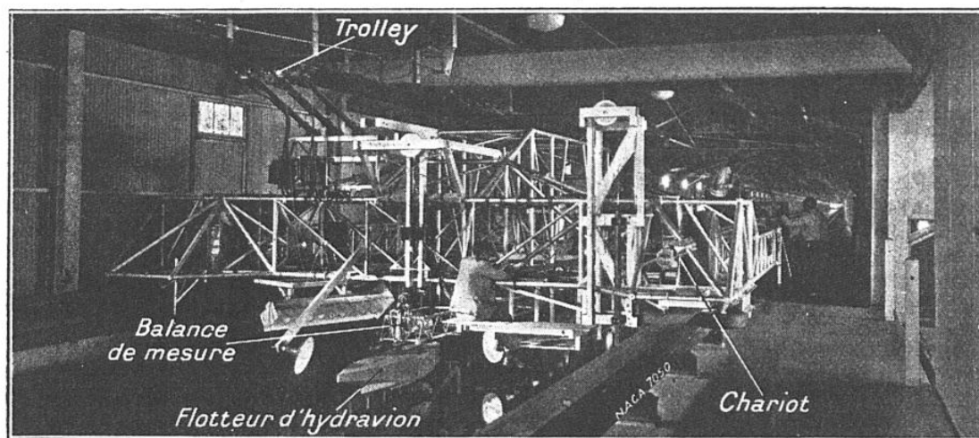
FIG. 6. — COMMENT ON ÉTUDIE LA FORME RATIONNELLE D'UN FLOTTEUR D'HYDRAVION FIXÉ SOUS LE CHARIOT DU BASSIN DES CARÈNES DU « N. A. C. A. » : LA VITESSE PEUT ATTEINDRE 130 KM/H ET LA LONGUEUR DU BASSIN DÉPASSE 870 MÈTRES
