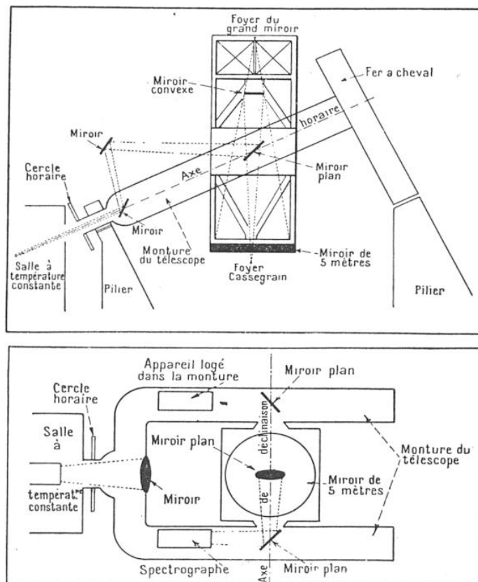
FIG. 8. — COUPE SCHÉMATIQUE ET VUE EN PLAN DU GRAND TÉLESCOPE DU MONT PALOMAR
