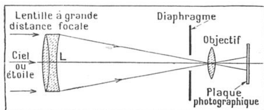
FIG. 2. — PHOTOMÈTRE PHOTOGRAPHIQUE POUR LE CIEL NOCTURNE
