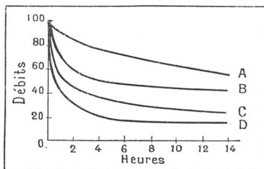
FIG. 6. — LA VARIATION DU DÉBIT D'HUILE A TRAVERS DIVERS GICLERS DE MÊME DIAMÈTRE DÉPEND DE LA NATURE DES MATÉRIAUX CONSTITUANT LES GICLERS. La courbe A se rapporte à un gicleur en verre ; B, à un gicleur en magnésium ; C, à un gicleur en laiton ; D, à un gicleur en fer pur ou acier. Tous ont 0,3 mm de diamètre.
