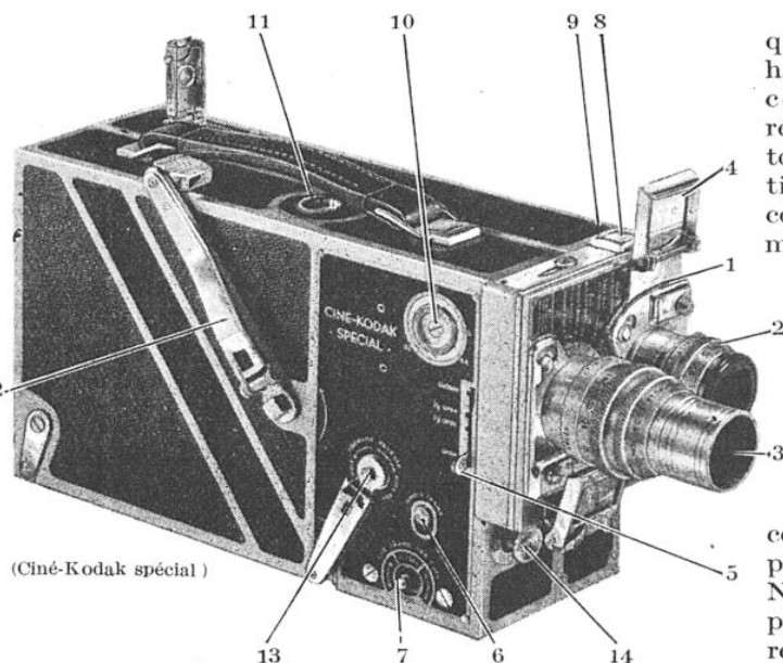
FIG. 6. — LE PLUS PERFECTIONNÉ DES APPAREILS CINÉMATOGRAPHIQUES DE FORMAT RÉDUIT
