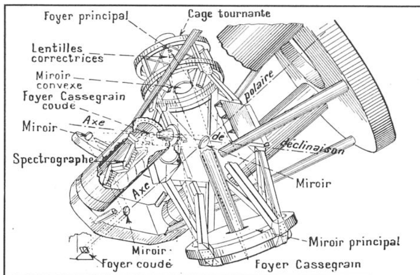
FIG. 9. — ENSEMBLE SCHÉMATIQUE DU TÉLESCOPE DE 5 MÈTRES DE DIAMÈTRE ET DE SA MONTURE, MONTRANT LA POSITION RESPECTIVE DES DIFFÉRENTS FOCYS OPTIQUES DE L'INSTRUMENT
