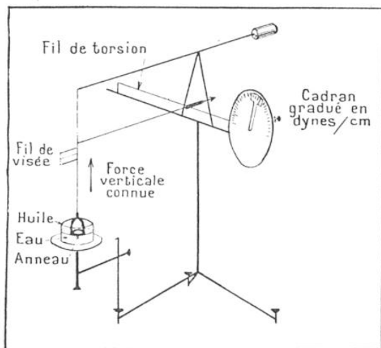
FIG. 8 ET 9. — SCHÉMA DE LA BALANCE « INTERFACIALE » POUR LA DÉTERMINATION DE LA TENSION SUPERFICIELLE DE L'EAU EN CONTACT AVEC L'HUILE, ET PHOTOGRAPHIE DE L'APPAREIL DE M. TRILLAT POUR L'ENREGISTREMENT AUTOMATIQUE DE CETTE TENSION EN FONCTION DU TEMPS
