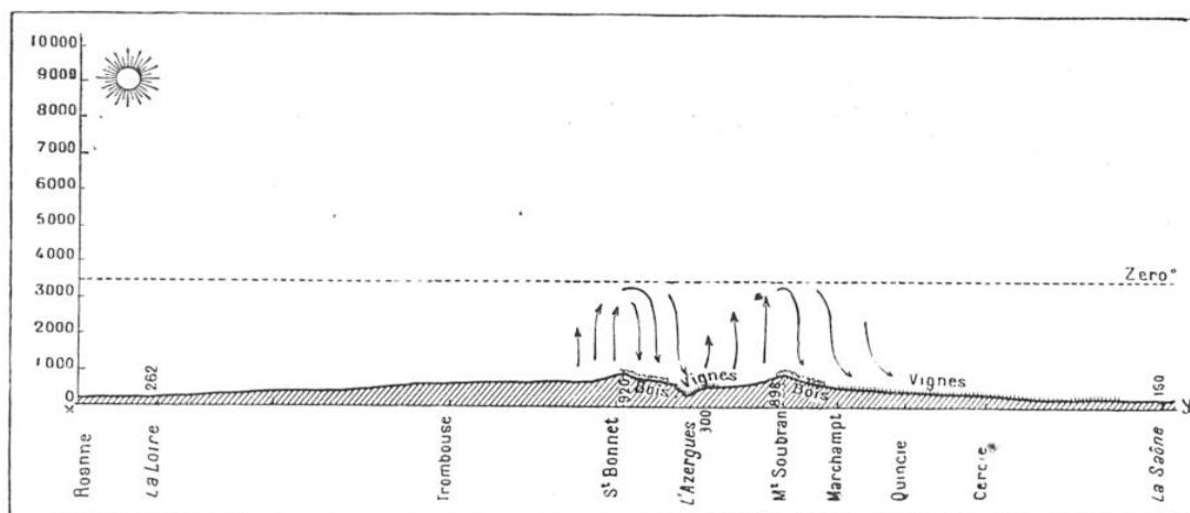
FIG. 4. — LES MOUVEMENTS ASCENDANTS DE L'AIR CHAUD ET HUMIDE PAR UNE BELLE JOURNÉE D'ÉTÉ, VERS 15 HEURES, SUR LES MONTS DU BEAUJOLAIS
