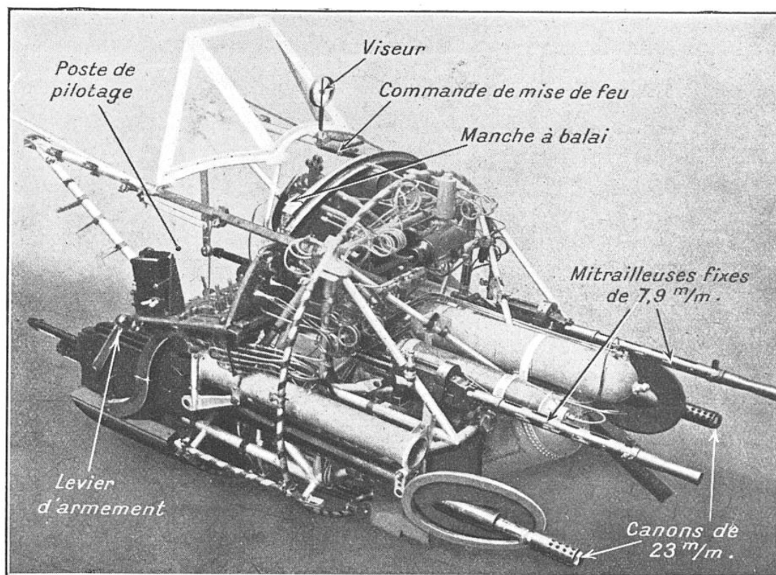
FIG. 3. — CE QUE CACHE UN FUSELAGE D'AVION D'ASSAUT
