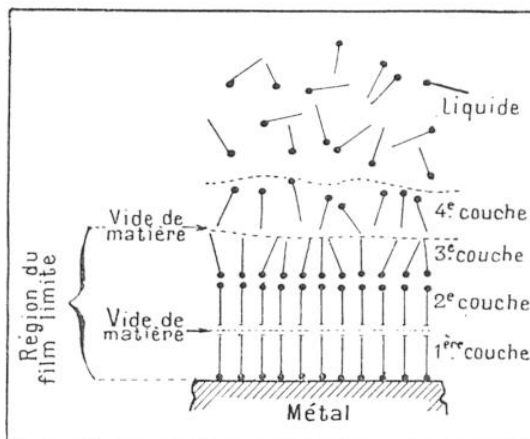
FIG. 3. — COMMENT S'ORIENTENT LES MOLECULES D'ACIDES GRAS AU VOISINAGE D'UNE SURFACE MÉTALLIQUE
