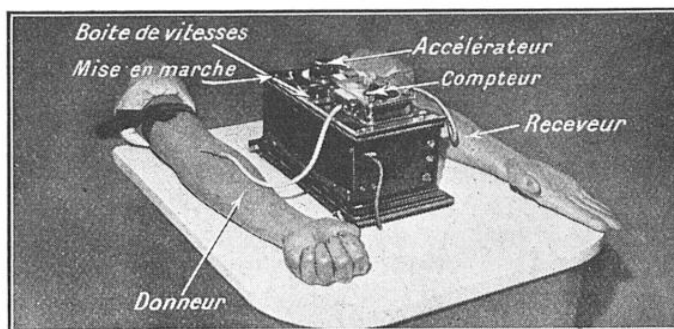
FIG. 10. — L'APPAREIL AUTOMATIQUE DE JOUVELET Il comporte un système moteur électrique intérieur, qui actionne une pompe curieuse dont le principe est expliqué figure 9. La vitesse d'écoulement est à la disposition de l'opérateur. Un compteur lui indique les doses transfusées à chaque instant.
