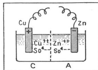
FIG. 3. — LA PILE DANIELL ET L'OXYDORÉDUCTION
