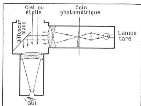
FIG. 1. — PHOTOMÈTRE VISUEL DE FABRY ET BUISSON (MODIFIÉ PAR DUFAY) POUR L'ÉTUDE DE LA LUMIÈRE DU CIEL NOCTURNE
