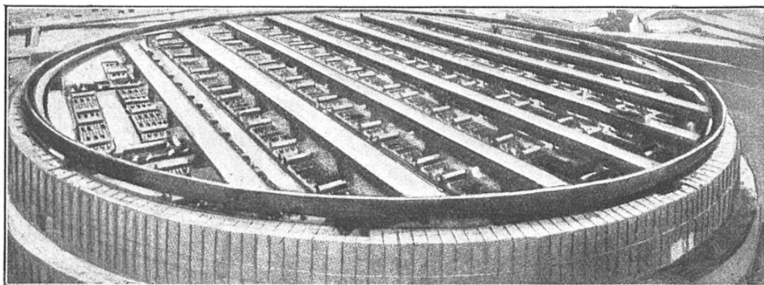
FIG. 5. — PARTIE INFÉRIEURE DU FOUR À RECUIRE LE BLOC DE « PYREX » DU MIROIR Cet immense plateau circulaire, sur lequel reposait le miroir, portait des séries de radiateurs électriques commandés automatiquement par des thermostats. La partie supérieure du four, portant un équipement analogue, s'emboîtait exactement sur ce plateau de base. La température à l'intérieur du four était abaissée très lentement, à raison de 1 degré par jour. Le refroidissement a duré onze mois.
