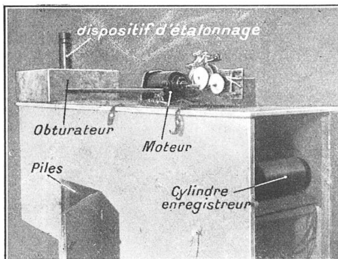
FIG. 7. — ENREGISTREUR PHOTOÉLECTRIQUE POUR L'ÉTUDE DES VARIATIONS DE LA LUMIÈRE DU CIEL NOCTURNE
