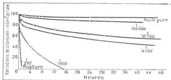
FIG. 10. — COMMENT VARIE, AVEC LE TEMPS, LA TENSION SUPERFICIELLE ENTRE EAU ET HUILE SUIVANT LA NATURE DE L'HUILE
