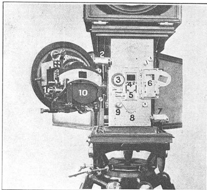
FIG. 2. — LE « SUPER-PARVO » OUVERT POUR LAISSER VOIR LES DIFFÉRENTS MÉCANISMES ASSURANT L'OBTURATION ET L'ENTRAÎNEMENT DU FILM
