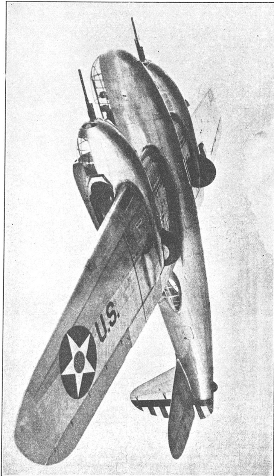
FIG. 4. — LE PLUS PUISSANT AVION D'ASSAUT CONSTRUIT JUSQU'ICI DANS LE MONDE : LE « BELL XFM-1 », MOTEUR ALLISON « V-1710 » Construit par la Bell Aircraft Co, de Buffalo (Etats-Unis), cet avion est mû par deux moteurs Allison (production de la General Motors) de 1 000 ch chacun, à deux cylindres en V, turbo-compresseur, refroidissement par l'éthyl-glycol. Il est armé de deux canons automatiques de 37 mm sur l'avant des moteurs et de deux tourelles en fuselage. Le 37 mm, à grande vitesse initiale et cadence élevée, permet un tir efficace à une distance de 1 500 à 2 000 m. On peut, dès lors, envisager pour cet appareil des missions assez différentes de celles qui sont confiées aux autres appareils d'assaut et qui ne comporteraient pas le vol à basse altitude. Telle serait l'attaque en piqué à 2 000 m, par des projectiles percutants à fusée instantanée, de batteries terrestres de D. C. A. ou des passerelles et des organes de D. C. A. non protégés des navires. Telle serait encore l'attaque des navires légers eux-mêmes, avec des obus de rupture qui pourraient aisément perfriser des blindages de 40 à 50 mm. Une rafale ajustée de trente à quarante projectiles, qu'il serait possible de tirer au cours d'une passe, serait extrêmement dangereuse pour le personnel et le matériel.
