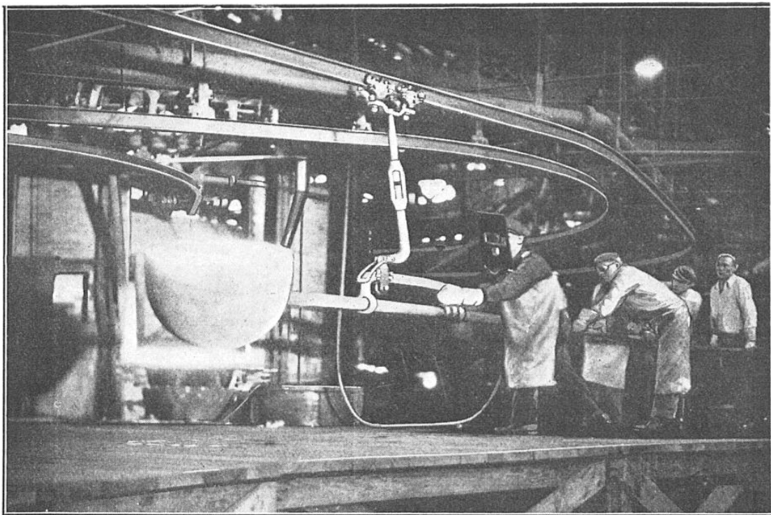
FIG. 2. — LE « PYREX » EST TRANSPORTÉ, DEPUIS LE FOUR DE FUSION DE 65 TONNES JUSQU'AU MOULE DU MIROIR, DANS D'ÉNORMES POCHES CONTENANT CHACUNE 350 KG DE VERRE FONDU ET SE DÉPLAÇANT SUSPENDUES À UN CHARIOT QUI ROULE SUR UN RAIL
