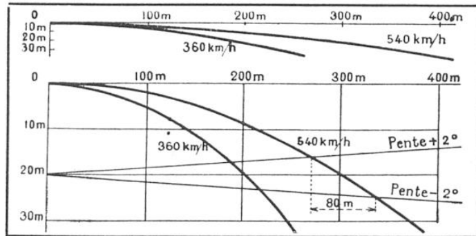
FIG. 1. — PORTÉES DE BOMBES LANCÉES EN VOL RASANT
