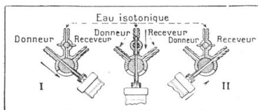
FIG. 8. — SCHÉMA DE FONCTIONNEMENT DE LA SERINGUE DU DOCTEUR TZANCK
