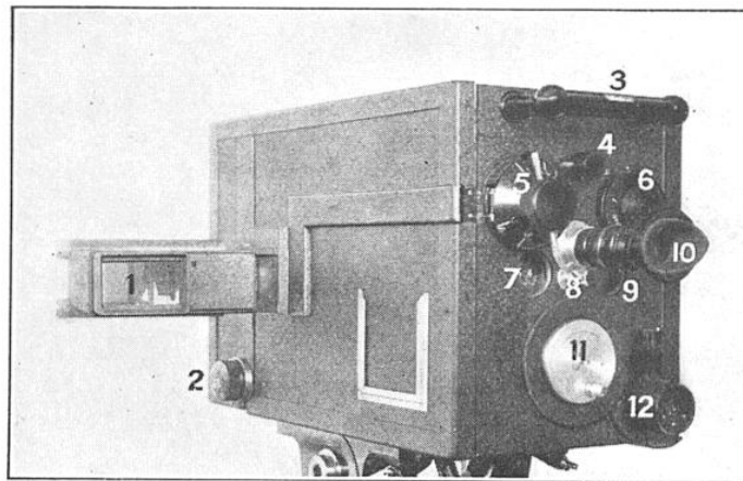
FIG. 1. — LES DIVERS ORGANES DE MANŒUVRE DU « SUPER-PARVO » (VU DU COTÉ OPPOSÉ À L'OBJECTIF) 1, viseur ; 2, bouton d'ouverture ; 3, niveau d'eau ; 4, « fondu » automatique ; 5, mise au point ; 6, bouton de diaphragme ; 7, compteur de mètres ; 8, clé de passage sur verre dépoli ; 9, indicateur de vitesse ; 10, loupe de visée ; 11, volant d'entraînement du mécanisme ; 12, conjoncteur et prise de courant.
