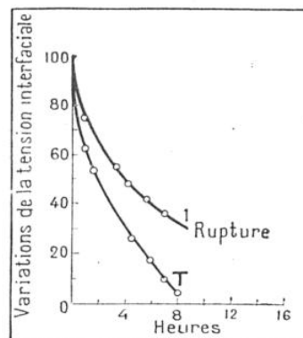
FIG. 11. — COMMENT VARIENT LES PROPRIÉTÉS D'UNE HUILE APRÈS CONTACT AVEC DES PIÈCES MÉTALLIQUES
