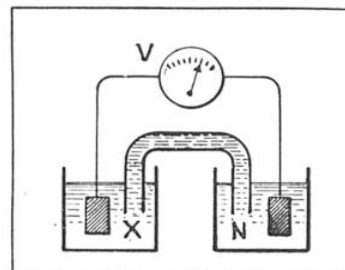
FIG. 1. — DISPOSITIF SCHÉMATIQUE POUR LA MESURE DU « pH »
