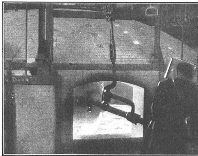
FIG. 3. — LE « PYREX » EN FUSION EST VERSÉ SUR LE MOULE EN BRIQUES DE CÉRAMIQUE RECOUVERTES DE POUDRE DE SILICE POUR EN ADOUCIR LES SURFACES. Le moule est surmonté d'un dôme isolant portant à sa surface interne des radiateurs électriques maintenant une température de 1\,350^{\circ} pendant la durée du remplissage.
