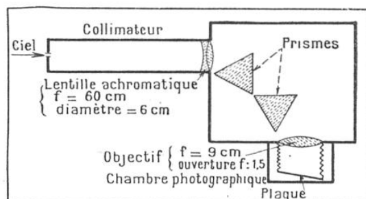
FIG. 3. — SPECTROGRAPHE POUR L'ÉTUDE DES RAIES ET DU SPECTRE CONTINU DE LA LUMIÈRE DU CIEL NOCTURNE
