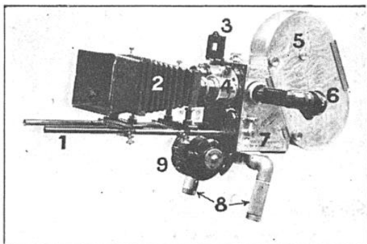
FIG. 4. — UN REMARQUABLE APPAREIL PORTATIF DE REPORTAGE CINÉMATOGRAPHIQUE
