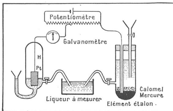
FIG. 2. — DISPOSITION PRATIQUE POUR LA MESURE DU « pH »
