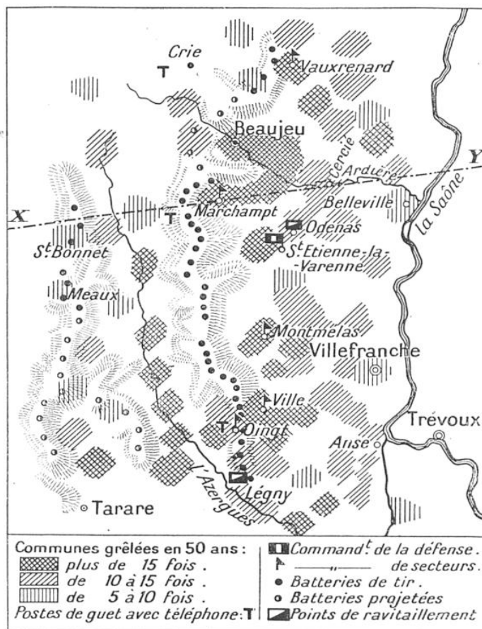
FIG. 3. — CARTE DES OPÉRATIONS DE LA LUTTE CONTRE LA GRÊLE PRATiquÉE EN 1936-1937 DANS LE BEAUJOLAIS La ligne marquée X-Y est celle suivant laquelle le terrain est supposé coupé dans les schémas détaillés des pages suivantes.
