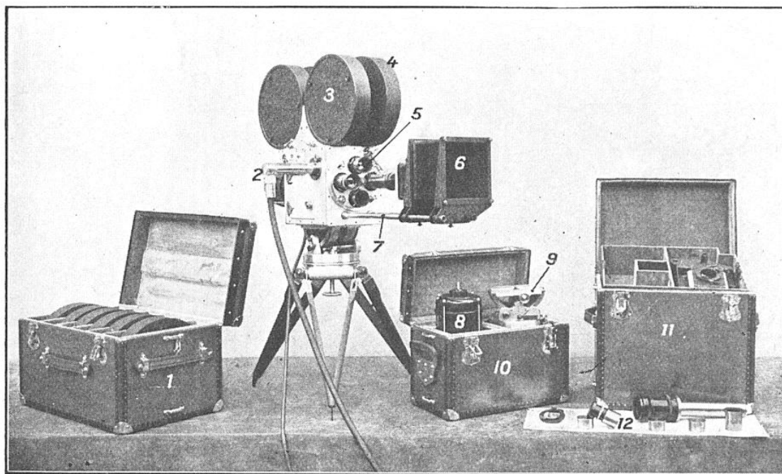
FIG. 3. — ENSEMBLE DE L'APPAREIL MIXTE « CAMERÉCLAIR », POUR LA PRISE DE VUES ET L'ENREGISTREMENT DU SON A L'EXTÉRIEUR, AVEC SES ACCESSOIRES
