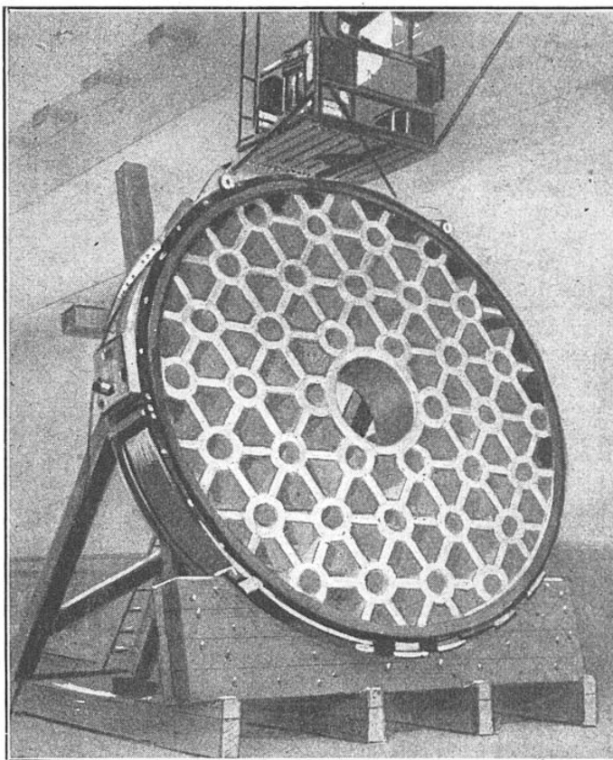
FIG. 7. — LE GRAND MIROIR DE 5 MÈTRES DE DIAMÈTRE PRÊT À ÊTRE EXPÉDIÉ, APRÈS COULAGE, À L'ATELIER DE TAILLE OPTIQUE. On remarque le cloisonnement cellulaire qui réduit le poids du miroir et assure un rapide équilibre de température entre ses diverses parties, condition essentielle pour obtenir des images nettes des astres éloignés.
