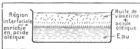
FIG. 7. — A LA SURFACE DE SÉPARATION DE L'EAU ET DE L'HUILE, LES MOLÉCULES GRASSES ACTIVES VIENNENT SE FIXER COMME A LA SURFACE D'UN MÉTAL
