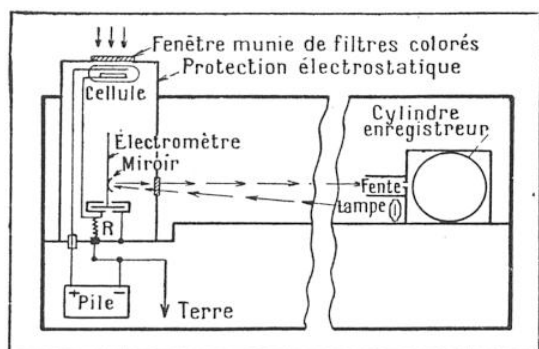
FIG. 4. — APPAREIL PHOTOÉLECTRIQUE ENREGISTREUR POUR L'ÉTUDE DE LA LUMIÈRE DU CIEL NOCTURNE
