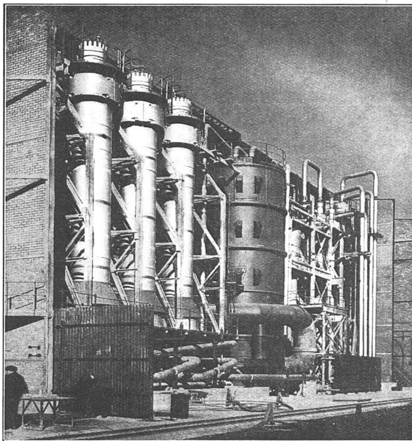
FIG. 2. — ENSEMBLE DE L'INSTALLATION D'HYDROGÉNATION EN PHASE LIQUIDE DE BILLINGHAM (ANGLETERRE)
