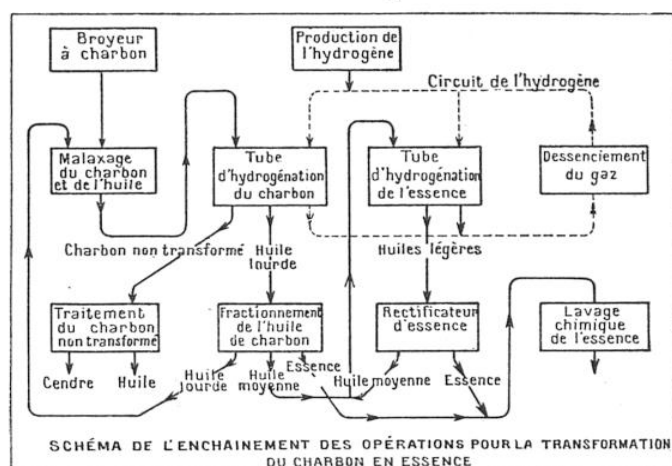
FIG. 7. — OPÉRATIONS SUCCESSIVES POUR LA FABRICATION DE L'ESSENCE PAR HYDROGÉNATION DU CHARBON
