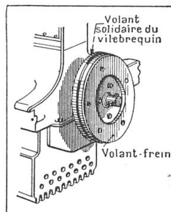
FIG. 11. — AMORTISSEUR DE TORSION DE LANCHESTER, OU « DAMPER », MONTÉ À L'AVANT DU VILEBREQUIN
