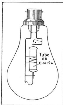
LAMPE A VAPEUR DE MERCURE SURPRESSÉE
