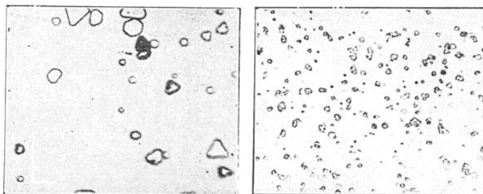
FIG. 8 ET 9. — MICROPHOTOGRAPHIES DE GRAINS PHOTOGRAPHIQUES SENSIBILISÉS A L'INFRAROUGE
