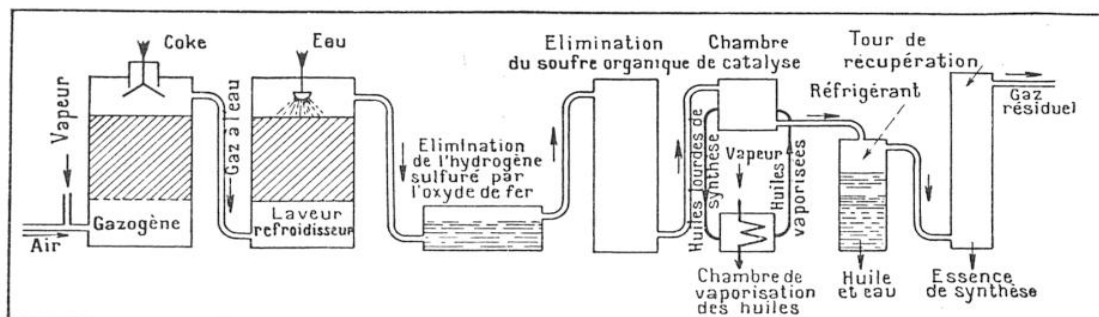
FIG. 11. — TABLEAU D'ENSEMBLE DU DISPOSITIF FISCHER-TROPSCH POUR LA FABRICATION DE L'ESSENCE SYNTHÉTIQUE À PARTIR DU GAZ À L'EAU
