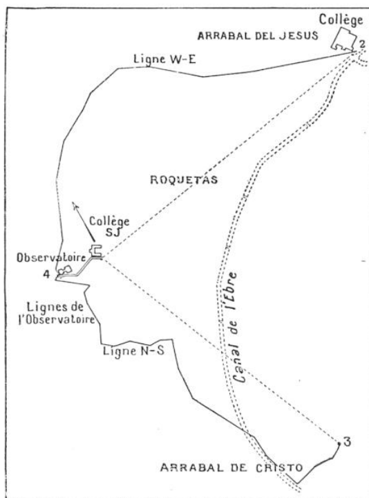
FIG. 1. — DISPOSITION DES LIGNES NORD-SUD ET EST-OUEST POUR L'ÉTUDE DES COURANTS TELLURIQUES A L'OBSERVATOIRE DE L'ÈBRE, PRÈS TORTOSA (ESPAGNE)
