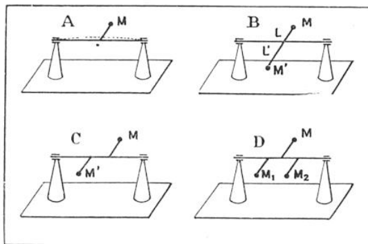
FIG. 1. — L'ÉQUILIBRAGE STATIQUE ET DYNAMIQUE DES MASSES EXCENTRÉES
