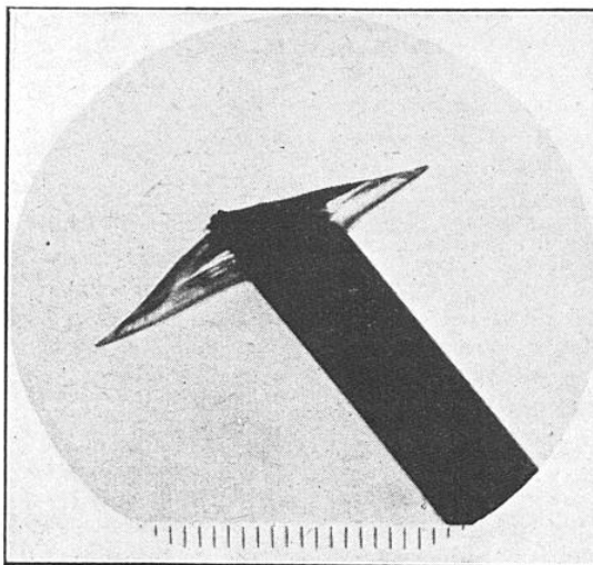
FIG. 8. — MICROSCALPEL FORMÉ D'UN ÉCLAT DE VERRE SOUDÉ À L'EXTRÉMITÉ D'UNE TIGE DE PLATINE (ÉCHELLE AU 1/100 MM)
