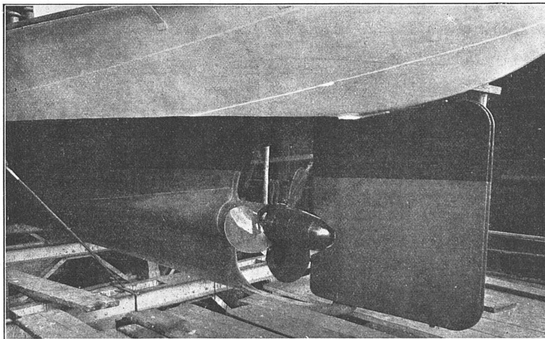
FIG. 3. — L'HÉLICE A PAS VARIABLE DE LA VEDETTE « ETZEL »
