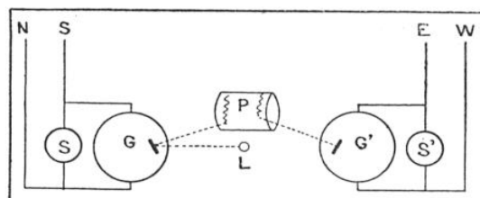
FIG. 4. — SCHÉMA DE L'ENREGISTREMENT DE COURANTS TELLURIQUES
