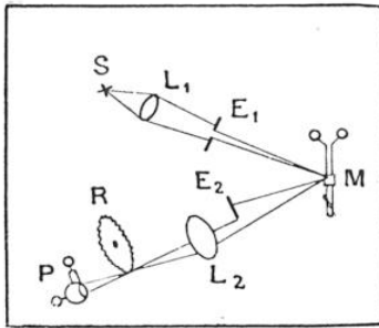
FIG. 3. — SCHÉMA DE PRINCIPE DE LA TRANSMISSION PAR MODULATION PAR TEMPS
