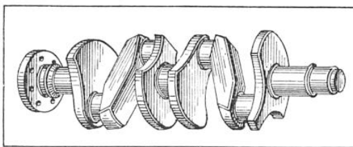
FIG. 5. — VILEBREQUIN D'UN MOTEUR A 4 CYLINDRES ET TROIS PALIERS AVEC SES CONTREPOIDS DE COMPENSATION
