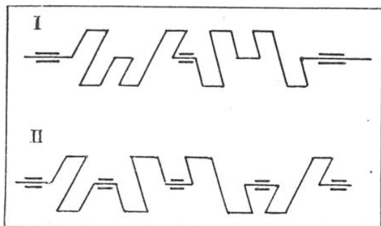
FIG. 7. — DEUX TYPES DE VILEBREQUINS POUR MOTEUR A 8 CYLINDRES
