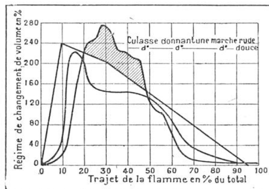
FIG. 12. — CES COURBES METTENT EN ÉVIDENCE LA VARIATION DANS L'ALLURE DE LA COMBUSTION POUR DEUX TYPES DE CULASSES. La courbe supérieure a été obtenue avec la même chambre de combustion que la courbe inférieure, mais avec une bougie écartée de 10 mm de son emplacement original. La deuxième donne un fonctionnement « doux », la première un fonctionnement « rude ». La ligne brisée représente la frontière entre les deux domaines à partir de laquelle commence la « rudesse du moteur » et les vibrations du carter.
