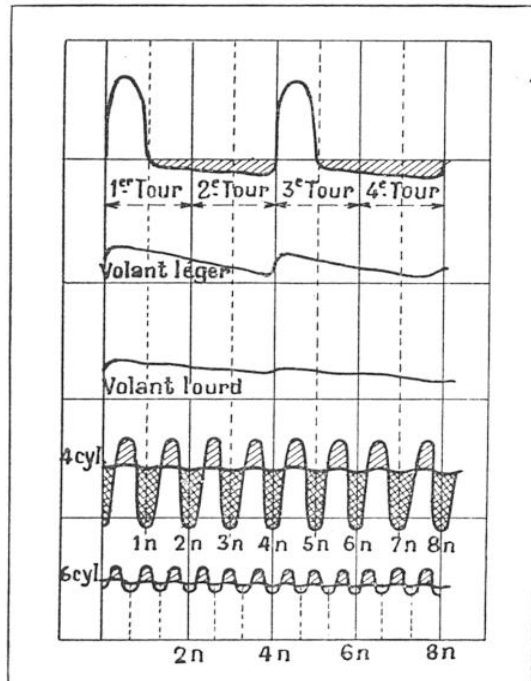
FIG. 10. — COMMENT VARIE LE COUPLE MOTEUR POUR DIVERS TYPES DE MOTEURS COMPORTANT 1, 4 ET 6 CYLINDRES
