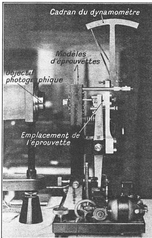
FIG. 10. — LA MICROMACHINE UTILISÉE PAR M. PORTEVIN POUR LES ESSAIS MÉCANIQUES DES MÉTAUX SUR ÉPROUVETTES RÉDUITES. La microéprouvette est fixée entre les mâchoires de la machine qui lui imposent un effort soit de traction, soit de cisaillement, jusqu'à rupture. L'effort supporté est mesuré au dynamomètre.
