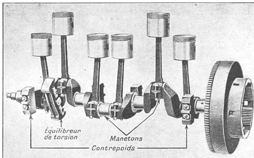
FIG. 6. — TYPE DE VILEBREQUIN D'UN MOTEUR A 6 CYLINDRES (BUICK) AVEC ÉQUILIBREUR DE TORSION ET CONTREPOIDS
