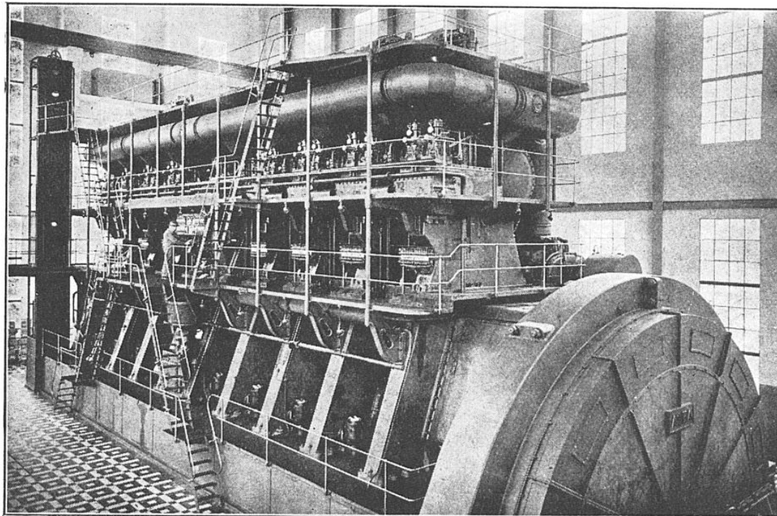
FIG. 3. — VUE D'ENSEMBLE DE L'UN DES TROIS MOTEURS DE 15 000 kW (22 000 ch) DE LA CENTRALE A MOTEURS DIESEL DE COPENHAGUE (DANEMARK)
