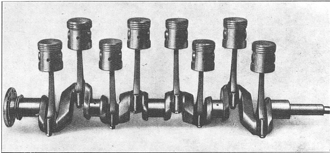
FIG. 9. — ENSEMBLE D'UN VILEBREQUIN AVEC PISTONS ET EMBIELLAGE DE MOTEUR A 8 CYLINDRES TYPE ÉQUILIBRÉ (VILEBREQUIN SANS CONTREPOIDS)
