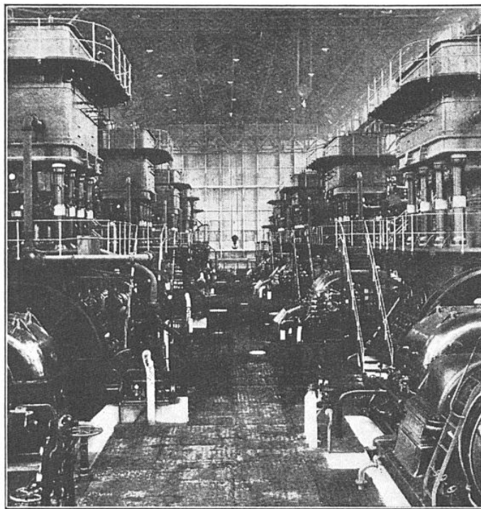
FIG. 9. — LA SALLE DES COMPRESSEURS D'HYDROGÈNE A MOYENNE ET A HAUTE PRESSION A L'USINE D'HYDROGÉNATION DE BILLINGHAM (ANGLETERRE)
