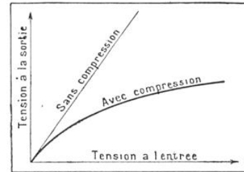
FIG. 6. — CARACTÉRISTIQUES D'UN AMPLIFICATEUR AVEC ET SANS DISPOSITIF DE COMPRESSION DES NUANCES
