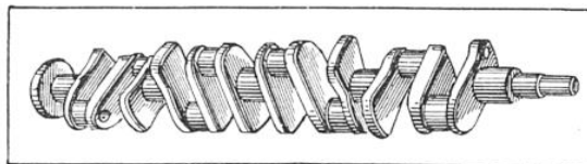
FIG. 8. — VILEBREQUIN DE MOTEUR A 8 CYLINDRES DU TYPE ÉQUILIBRÉ
