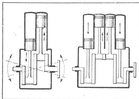
FIG. 3. — L'ÉQUILIBRAGE DES FORCES D'INERTIE ET DES COUPLES SUR LES MOTEURS A 2 ET A 4 CYLINDRES
