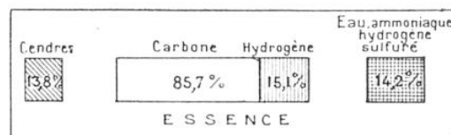
FIG. 5. — LES PRODUITS RÉSULTANT THÉORIQUEMENT DE L'HYDROGÉNATION DU CHARBON
