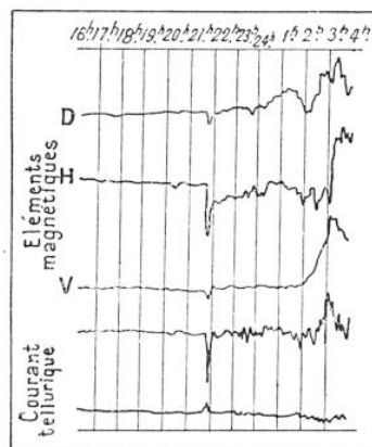
FIG. 7. — L'ENREGISTREMENT DES PHÉNOMÈNES INSTANTANÉS MONTRÉ QUE LE DÉBUT DES ORAGES MAGNÉTIQUES COÏNCIDE EXACTEMENT AVEC UNE VARIATION BRUSQUE DE L'INTENSITÉ DES COURANTS TELLURIQUES
