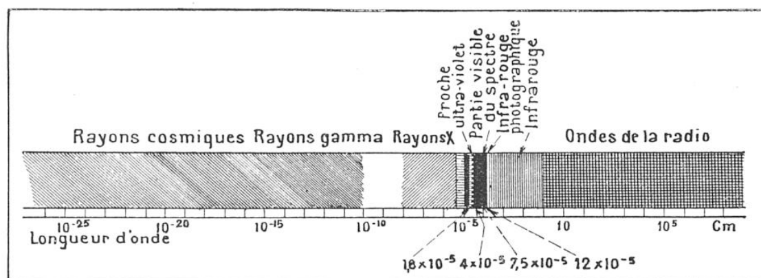
FIG. 2. — SPECTRE COMPLET DES RADIATIONS ÉLECTROMAGNÉTIQUES, DEPUIS LES ONDES LES PLUS LONGUES DE LA RADIOÉLECTRICITÉ JUSQU'ÀUX RAYONS COSMIQUES
