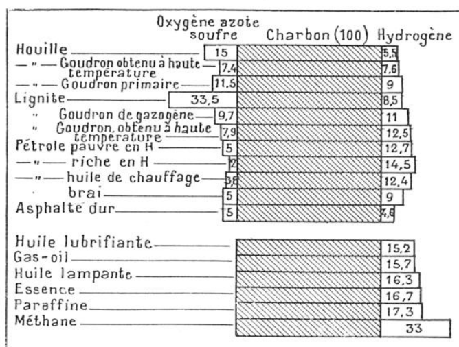
FIG. 4. — TENEUR EN HYDROGÈNE DE DIVERS COMBUSTIBLES : CHARBONS, GOUDRONS, HYDROCARBURES, ETC., RAPPORTÉE A 100 PARTIES DE CARBONE
