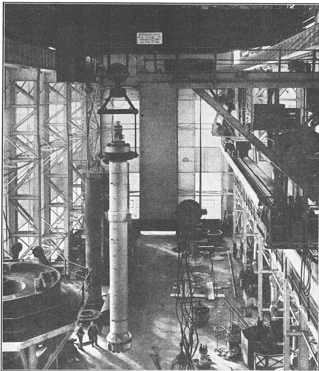
UN TUBE D'HYDROGÉNATION EN « PHASE LIQUIDE » AUX USINES DE BILLINGHAM (ANGLETERRE) POUR LA FABRICATION SYNTHÉTIQUE DES CARBURANTS
