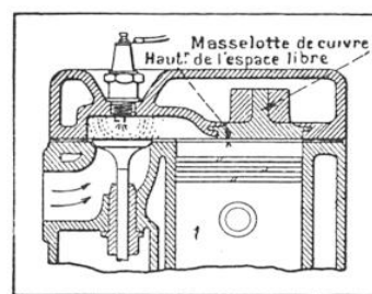
FIG. 14. — COUPE TRANSVERSALE D'UNE CULASSE COMPOSITE FONTE-CUIVRE
