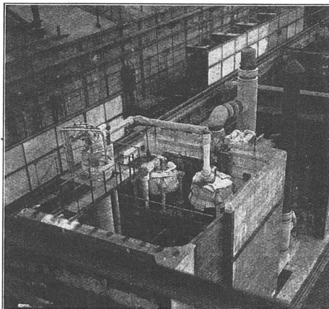
FIG. 1. — UNE UNITÉ D'HYDROGÉNATION A L'USINE DE LEUNA (ALLEMAGNE), LA PLUS IMPORTANTE DU MONDE. Les tubes de catalyse sont disposés dans des « blockhaus », en béton armé afin de limiter les risques d'explosion. Cette mesure de précaution a été reconnue superflue comme le montre la figure 2.
