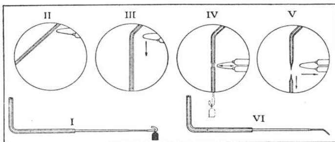
FIG. 6. — LES DIVERSES PHASES SUCCESSIVES DE LA FABRICATION D'UNE MICROPIPETTE EN VERRE
