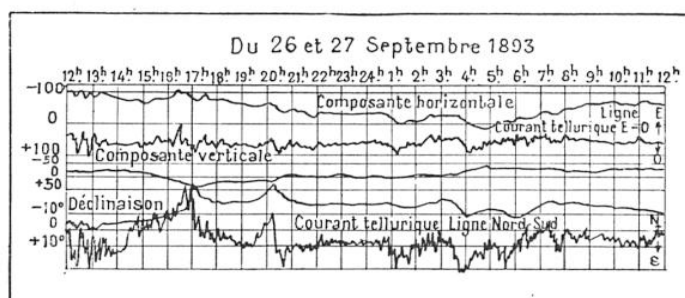
FIG. 8. — DIAGRAMME METTANT NETTEMENT EN ÉVIDENCE LES RELATIONS ENTRE LES COURANTS TELLURIQUES ET LES COMPOSANTES DU MAGNÉTISME TERRESTRE. Ces courbes, relevées par les services telluriques permanents du Parc-Saint-Maur, montrent le parallélisme frappant entre les variations moyennes du courant tellurique Est-Ouest et la force magnétique horizontale, d'une part, du courant tellurique Nord-Sud et de la déclinaison d'autre part.
