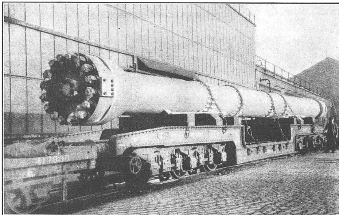
FIG. 6. — TUBE D'HYDROGÉNATION A HAUTE PRESSION, FABRIQUÉ EN ANGLETERRE POUR L'ITALIE, EN VUE DU TRAITEMENT DE LIGNITES, DE SCHISTES ET DES PÉTROLES D'ALBANIE
