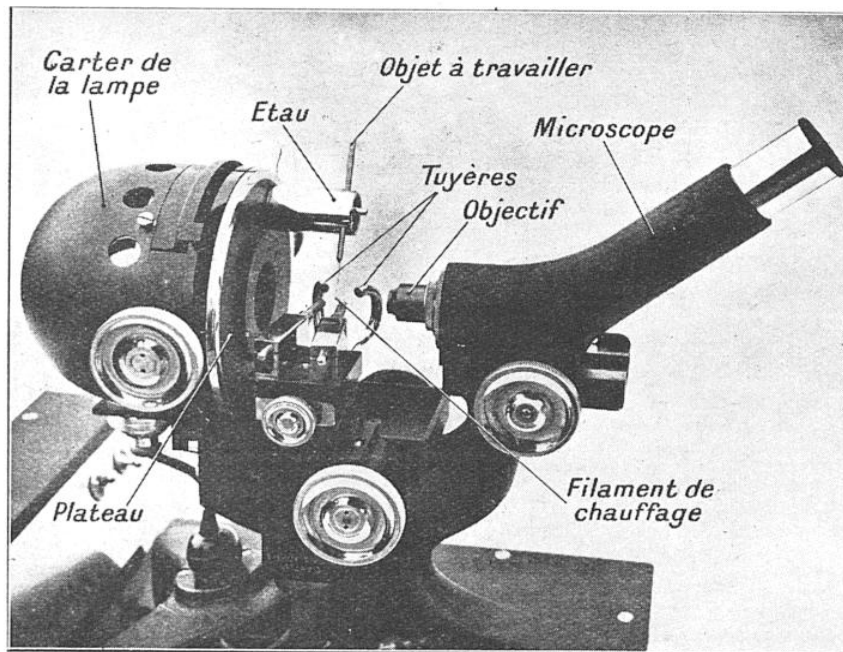
FIG. 5. — DÉTAILS DES DIFFÉRENTS ORGANES DE LA MICROFORGE UTILISÉE POUR LA FABRICATION DES MICROOUTILS
