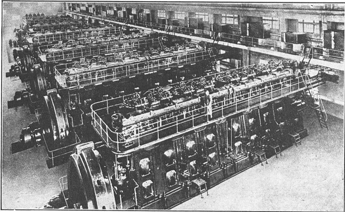
FIG. 5. — VUE GÉNÉRALE DE LA NOUVELLE CENTRALE DE SHANGHAI (CHINE), ÉQUIPÉE DE MOTEURS DIESEL D'UNE PUISSANCE TOTALE D'ENVIRON 50 000 CH
