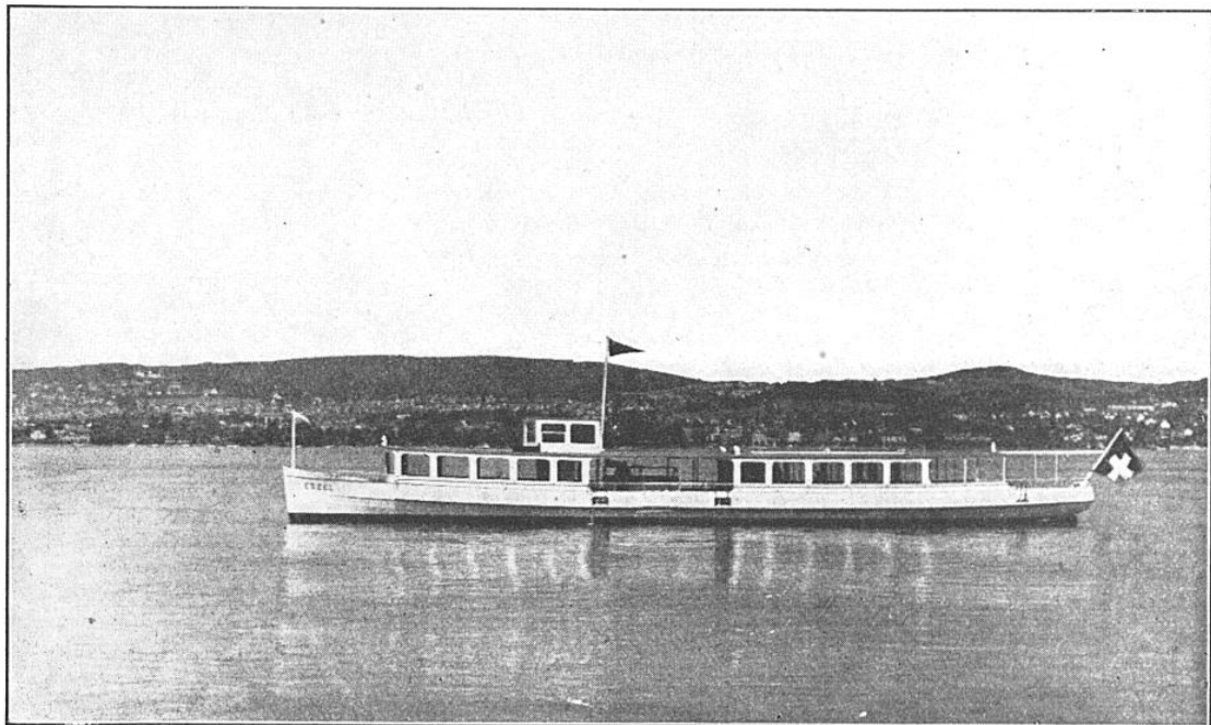
FIG. 1. — LA VEDETTE « ETZEL », MUNIE D'UNE HÉLICE A PAS VARIABLE, SUR LE LAC DE ZURICH Ce bateau de 200 places environ, mû par un moteur Diesel de 250 ch, a accompli aujourd'hui 150 000 km et 80 000 manœuvres d'abordage en utilisant uniquement les propriétés de l'hélice à pas variable qui permet de changer très rapidement le sens de la marche et la vitesse du bâtiment.
