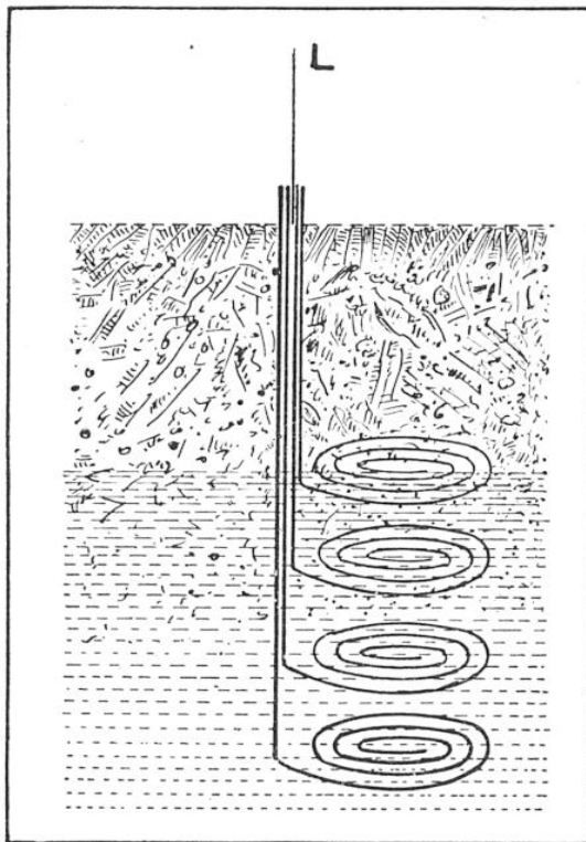
FIG. 2. — TYPE DE PRISE DE TERRE DE L'OBSERVATOIRE DU PARC-SAINT-MAUR, QUI DUT ÊTRE DÉPLACÉ PAR SUITE DE L'IMPORTANCE DES COURANTS INDUSTRIELS TRANSMIS PAR LE SOL DANS LA RÉGION PARISIENNE. Aux extrémités des lignes N.-S. et E.-W., le fil s'arrêtait à un poteau télégraphique et était relié à quatre couronnes ou spirales de fer galvanisé, de 4 mm de diamètre et de 30 m de longueur chacune, espacées verticalement de 50 cm et enfouies dans le sol entre 1 m et 2 m 50 de profondeur. L'espace entre les couronnes était rempli par des couches alternées de terre et de charbon de bois pulvérisé.
