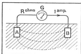
FIG. 3. — COMMENT ON EFFECTUE EN PRINCIPE LA MESURE D'UN COURANT TELLURIQUE
