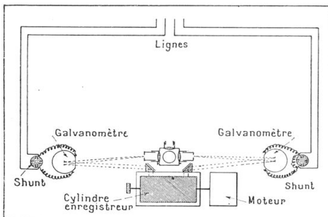
FIG. 5. — INSTALLATION POUR L'ENREGISTREMENT SIMULTANÉ, A L'OBSERVATOIRE DE L'ÈBRE (ESPAGNE), DES COURANTS TELLURIQUES N.-S. ET E.-W.
