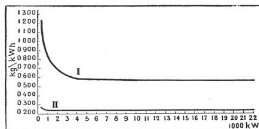
FIG. 2. — COURBES DE LA CONSOMMATION DE COMBUSTIBLE PAR kWh D'UNE CENTRALE A VAPEUR (I) ET D'UNE CENTRALE A MOTEURS DIESEL (II)
