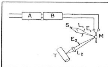
FIG. 5. — SCHÉMA DU DISPOSITIF DE RÉCEPTION DE L'IMAGE
