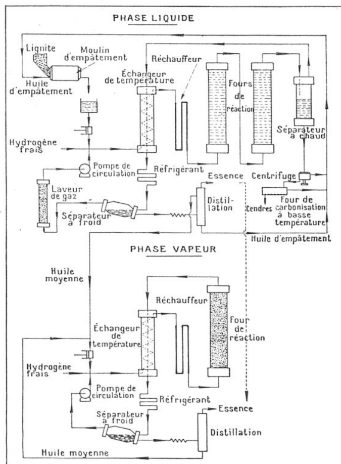
FIG. 8. — TABLEAU D'ENSEMBLE DES OPÉRATIONS EN PHASE LIQUIDE ET EN PHASE VAPEUR POUR L'OBTENTION D'ESSENCE PAR HYDROGÉNATION DU LIGNITE
