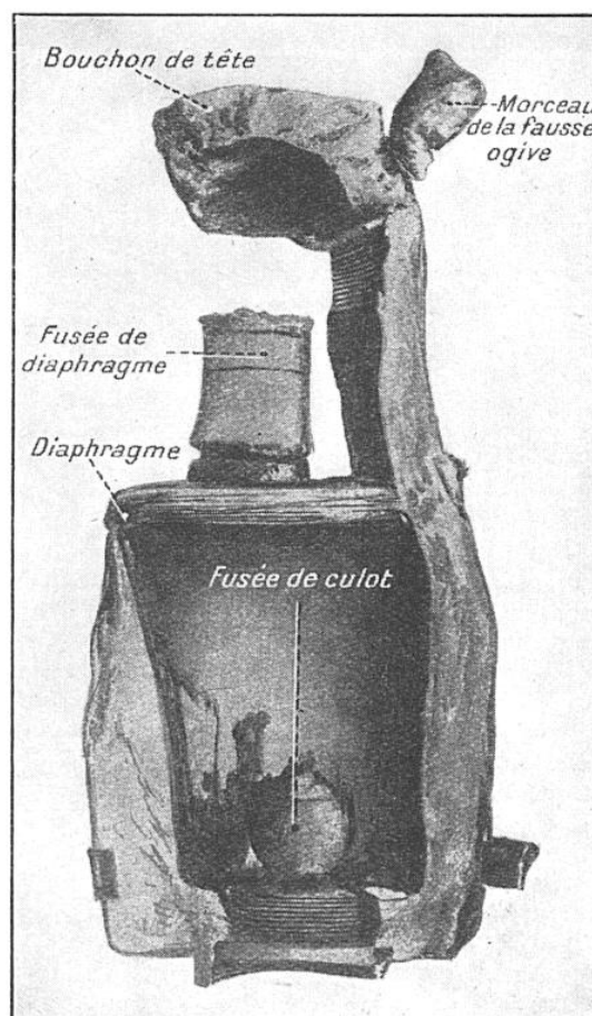
FIG. 2. - CE FRAGMENT D'OBUS DE LA « GROSSE BERTHA » A PERMIS DE RECONSTITUER LA FORME ET LES DÉTAILS DU PROJECTILE
