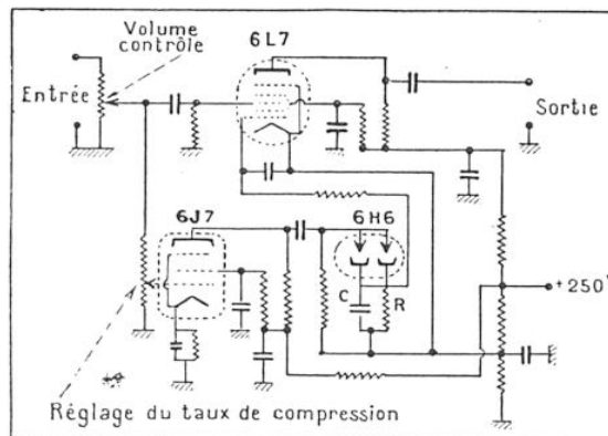
FIG. 7. — SCHÉMA D'UN AMPLIFICATEUR AVEC COMPRESSEUR DE NUANCES
