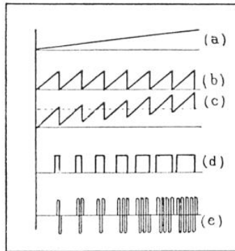
FIG. 4. — FORMES DES DIFFÉRENTES TENSIONS EXCITANT LE GALVANOMÈTRE
