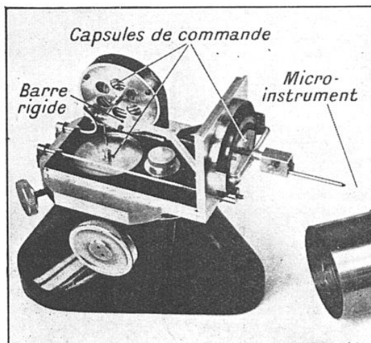
FIG. 4. — DÉTAILS DU MÉCANISME DU RÉCEPTEUR PORTANT LE MICROOUTIL
