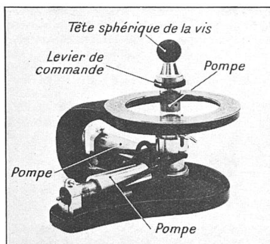
FIG. 3. — LE MICROMANIPULATEUR A ROTULE POUR LA COMMANDE DES MICROOUTILS DANS LE CHAMP DU MICROSCOPE
