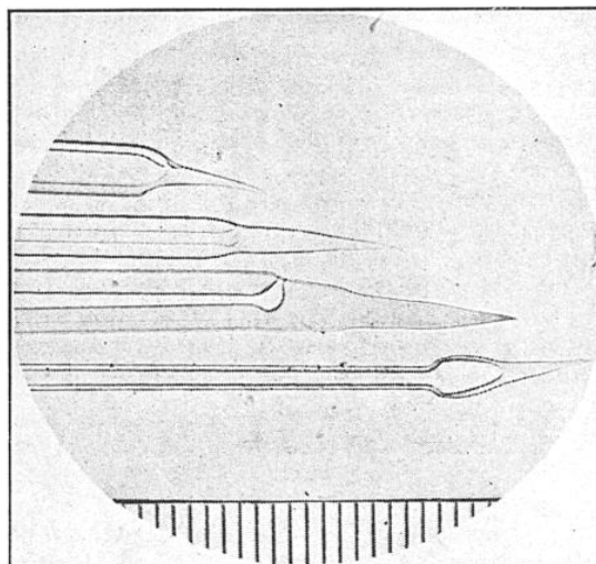
FIG. 7. — DIFFÉRENTS MODÈLES DE MICROPIPETTES EN VERRE SOUFFLÉ TERMINÉES PAR DES POINTES PLEINES TRÈS RÉSISTANTES. Chaque graduation indiquée sur l'échelle inférieure correspond à une longueur de 1/100 mm.
