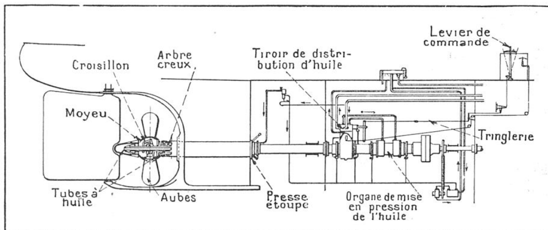
FIG. 2. — DISPOSITION SCHÉMATIQUE DE LA COMMANDE DE L'HÉLICE À PAS VARIABLE
