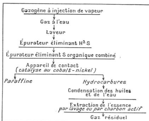
FIG. 10. — LES DIVERSES OPÉRATIONS SUCCESSIVES DE LA SYNTHÈSE DE L'ESSENCE PAR LE PROCÉDÉ FISCHER
