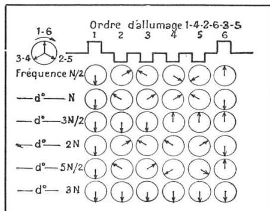
FIG. 13. — SCHÉMA DONNANT LA DIRECTION ET LE SENS DES FORCES D'INERTIE AUX DIFFÉRENTES HARMONIQUES POUR UN VILEBREQUIN DE 6 CYLINDRES
