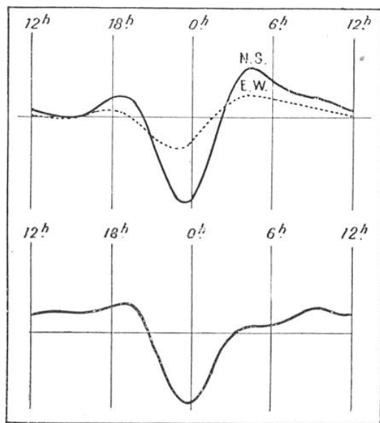
FIG. 6. — COURBES MOYENNES DU COURANT TELLURIQUE (EN HAUT) ET DU CHAMP MAGNÉTIQUE TERRESTRE TOTAL (EN BAS) ENREGISTRÉS A BERLIN, D'APRÈS WEINSTEIN
