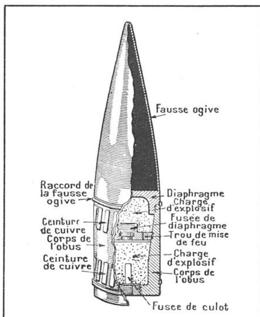
FIG. 1. — COUPE D'UN OBUS DE LA « BERTHA » Munis d'une fausse ogive, les obus — dont le calibre passait de 21 à 23,5 cm pour tenir compte de l'usure de la pièce au cours des soixante-cinq coups qu'elle devait tirer — pesaient de 100 à 115 kg et leur longueur variait de 0,90 m à 1,11 m. Ils étaient munis de deux fusées afin d'éviter tout raté d'éclatement, un projectile non éclaté pouvant fournir d'utiles renseignements à l'armée française.
