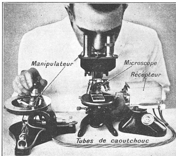
FIG. 1. — ENSEMBLE DU MICROMANIPULATEUR PNEUMATIQUE QUI PERMET AU SAVANT D'INTERVENIR SUR LA PLATINE DU MICROSCOPE
