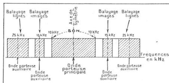
FIG. 3. — LA MODULATION COMPLEXE DE L'ONDE PORTEUSE DU SON DANS LE SYSTÈME DE TÉLÉVISION DU MONT
