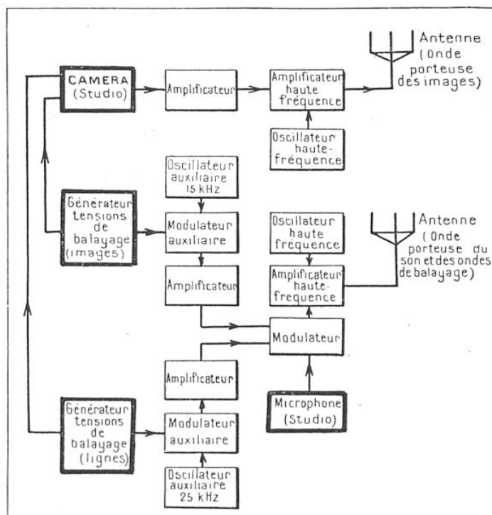
FIG. 4. — DISPOSITION SCHÉMATIQUE DES ORGANES DE L'ÉMETTEUR DANS LE SYSTÈME DU MONT
