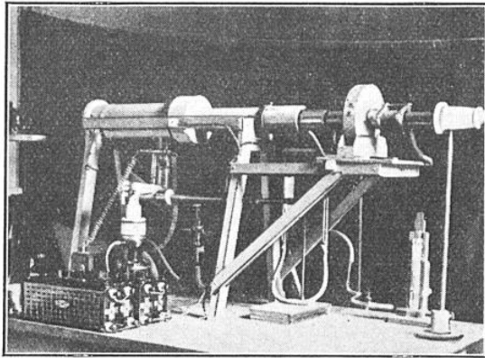
FIG. 4 — PHOTOGRAPHIE D'ENSEMBLE D'UN MICROSCOPE ÉLECTRONIQUE MAGNÉTIQUE
