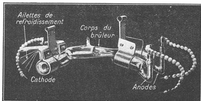
FIG. 3. — AUTRE TYPE DE BRULEUR EN QUARTZ POUR LA PRODUCTION DE RAYONS ULTRAVIOLETS
