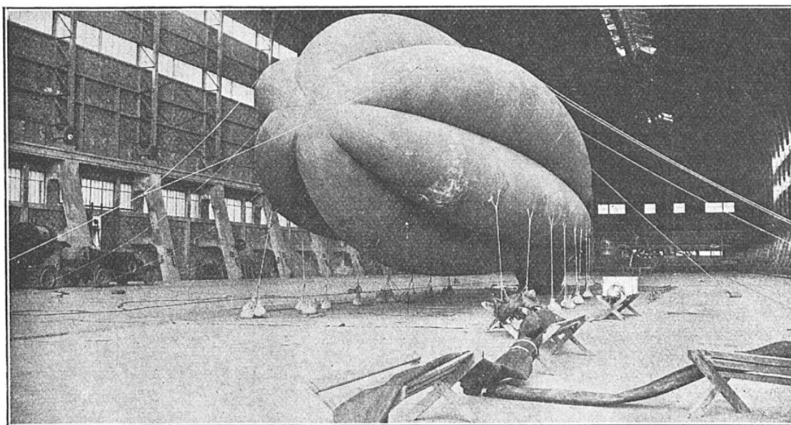
FIG. 5. — VUE D'ENSEMBLE D'UN BALLON A SIX LOBES AU HANGAR (ARIEL)
