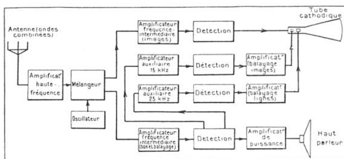
FIG. 5. — DISPOSITION SCHÉMATIQUE DES ORGANES D'UN RÉCEPTEUR DANS LE SYSTÈME DU MONT
