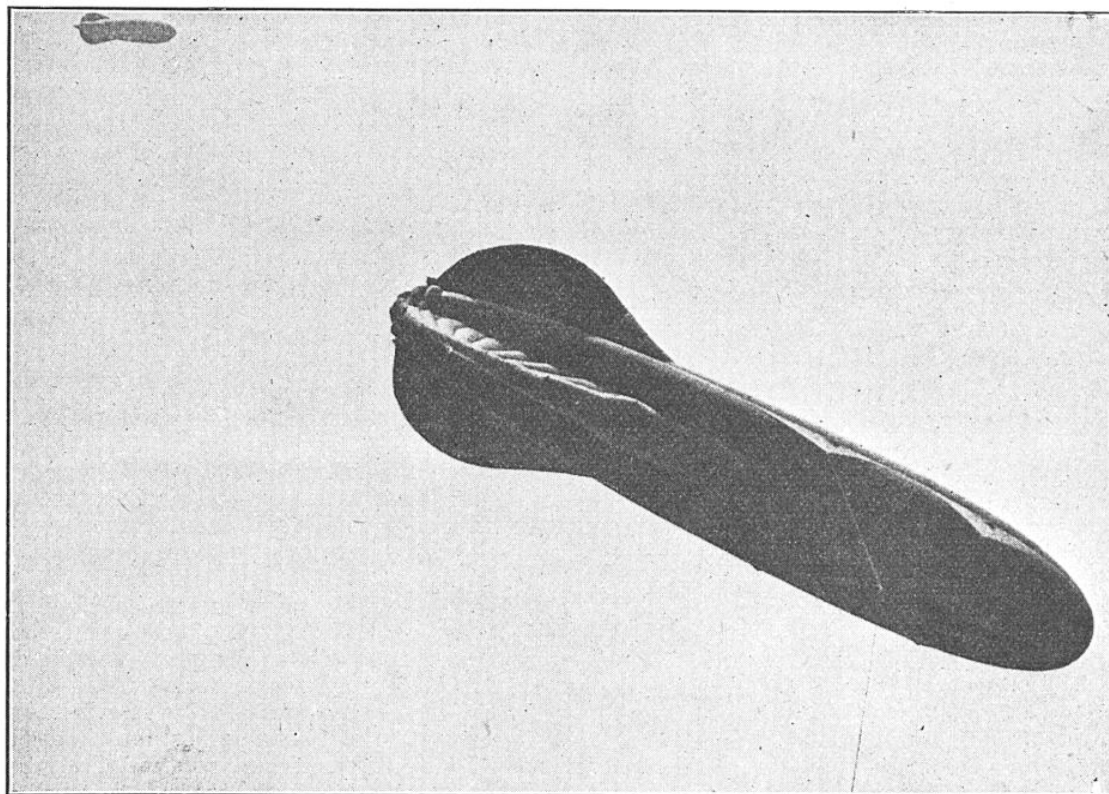
FIG. 3. — BALLON CAPTIF A LOBES AUTOSTABLE, SYSTÈME DU COMMANDANT LETOURNEUR, MONTRANT A L'ARRIÈRE LES EMPENNAGES A GONFLEMENT AÉRODYNAMIQUE
