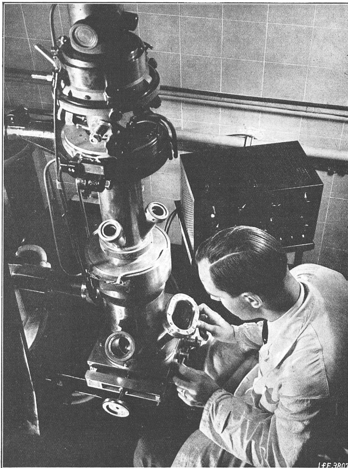
FIG. 13. — ENSEMBLE DU SUPERMICROSCOPE ÉLECTRONIQUE « SIEMENS ET HALSKE » QUI UTILISE DES TENSIONS DE L'ORDRE DE 100 000 VOLTS ET PERMET D'OBTENIR DES GROSSISSEMENTS VOISINS DE 20 000 FOIS, SOIT ENVIRON 10 FOIS PLUS QUE LE MEILLEUR MICROSCOPE OPTIQUE
