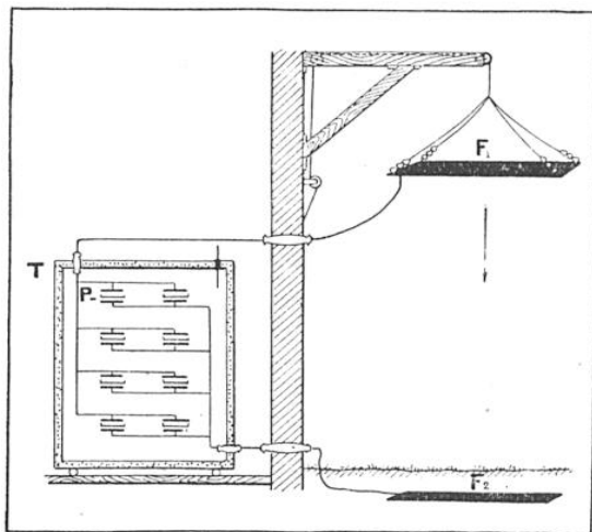
FIG. 3. — SCHÉMA DU MONTAGE ÉLECTRIQUE POUR L'ÉTUDE DE L'ACTION DE L'ÉLECTRICITÉ ATMOSPHÉRIQUE SUR LES MICROORGANISMES. La feuille métallique F_1 , de hauteur variable, est recouverte d'un mélange de bromures de sodium et de baryum. La feuille F_2 est mise à la terre. Dans le thermostat isolé T sont placées des boîtes de Pétri P contenant les cultures, entre deux disques métalliques.
