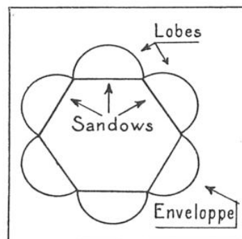
FIG. 2. — COUPE TRANSVERSALE D'UN BALLON A SIX LOBES MONTRANT LA DISPOSITION DES SANDOWS SUIVANT UN HEXAGONE
