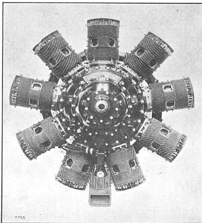
FIG. 4. — MOTEUR ANGLAIS SANS SOUPAPES « BRISTOL PERSEUS » A REFROIDISSEMENT PAR AIR
