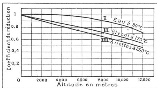
FIG. 5. — RÉDUCTION DE LA PUISSANCE DE REFOUDDISEMENT EN ALTITUDE
