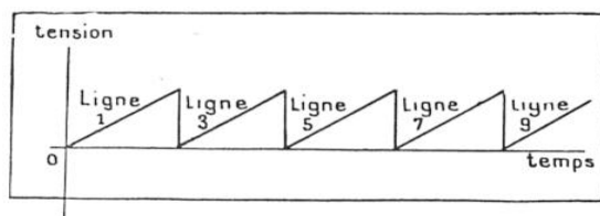
FIG. 2. — EXEMPLE TYPE D'UNE TENSION EN « DENTS DE SCIE » FOURNIE PAR UN GÉNÉRATEUR DE « TENSIONS DE BALAYAGE » (1) Lorsque la tension appliquée aux plaques de déviation de l'oscillographe cathodique croît de zéro à son maximum, le spot lumineux décrit une ligne de gauche à droite. Un générateur analogue fournit la tension appliquée à un deuxième groupe de plaques de déviation et provoque le déplacement des lignes de haut en bas. Les lignes d'exploration sont numérotées ici d'après le système d'entrelacement actuellement appliqué (demi-image impaire).
