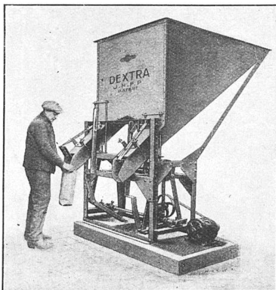
FIG. 7. — DOSEUSE A VOLUME CONSTANT POUR LE REMPLISSAGE DE SACS OU DE PAQUETS DE 5 A 50 LITRES
