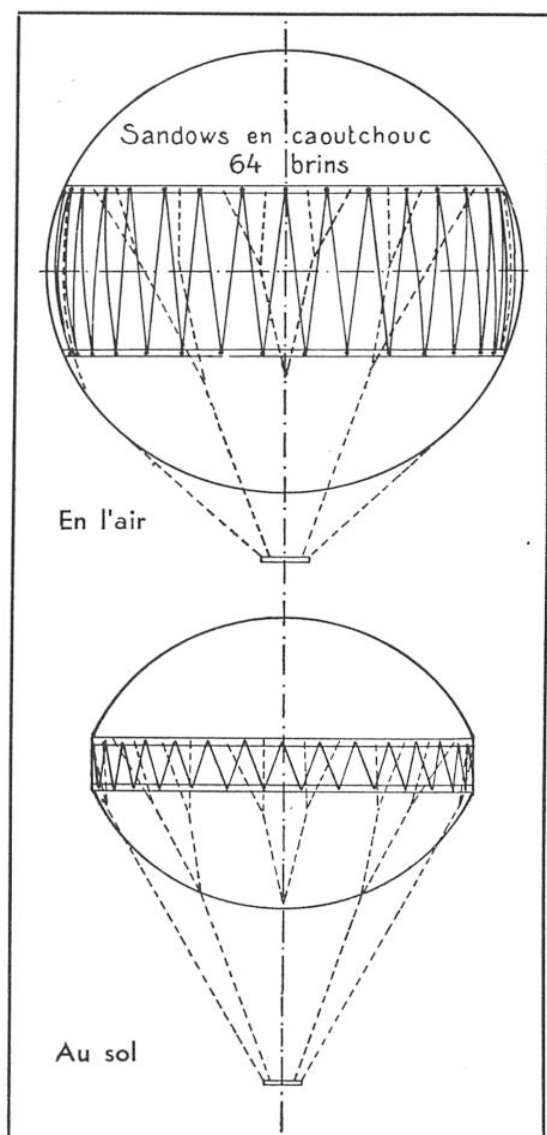
FIG. 1. — BALLON SPHÉRIQUE DILATABLE UTILISÉ PAR LES AÉROSTIERS ITALIENS Peu gonflé au sol, il se dilate en l'air.
