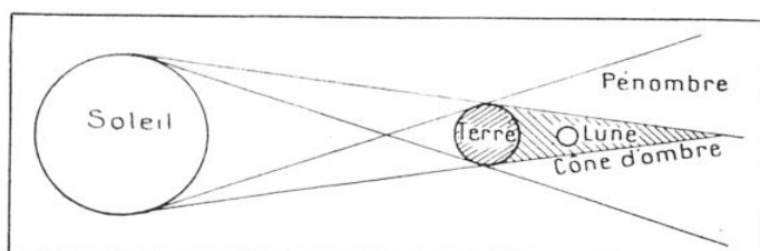
FIG. 1. — COMMENT SE PRODUIT UNE ÉCLIPSE DE LUNE
