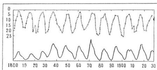
FIG. 16. — UNE CURIEUSE JUSTIFICATION SCIENTIFIQUE DE LA PRÉVISION DES ÉPIDÉMIES PAR L'ASTROLOGIE.
