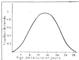
FIG. 6. — COURBE DONNANT LA FRACTION DE LA LUNE ÉCLAIRÉE PAR LE SOLEIL EN FONCTION DE L'ÂGE DE NOTRE SATELLITE
