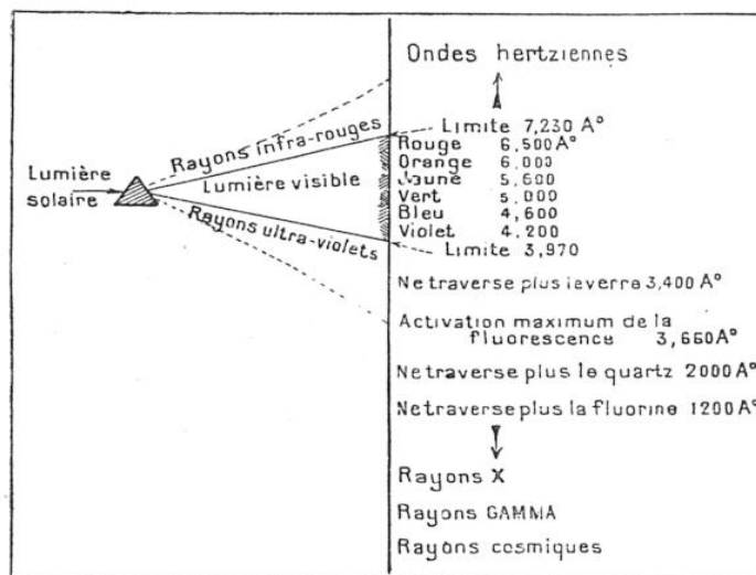
FIG. 1. — LA DÉCOMPOSITION DE LA LUMIÈRE SOLAIRE ET LA GAMME DES DIVERSES RADIATIONS DEPUIS LES ONDES HERTZIENNES JUSQU' AUX RAYONS COSMIQUES
