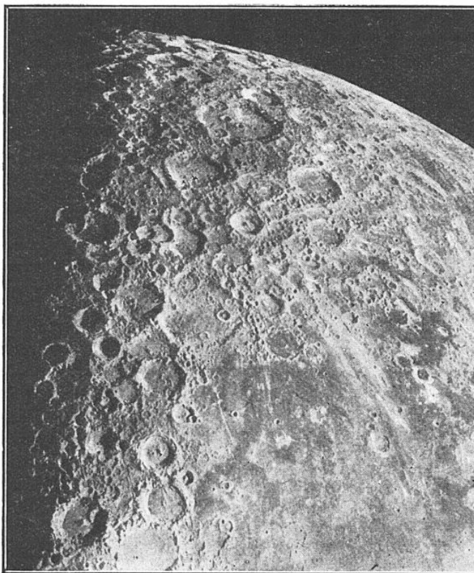
FIG. 4. — PHOTOGRAPHIE PARTIELLE DE LA LUNE OBTENUE A L'OBSERVATOIRE DU MONT WILSON
