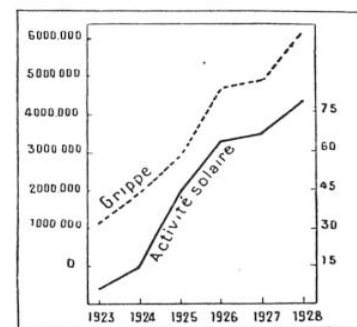
FIG. 8. — ACTIVITÉ SOLAIRE ET GRIPPE EN U. R. S. S. (DONNÉES ANNUELLES)
