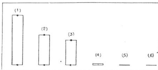
FIG. 16. — TABLEAU COMPARATIF DES POUVOIRS SÉPARATEURS DES MICROSCOPES, OPTIQUE ET ÉLECTRONIQUE, PAR RAPPORT AUX GRANDEURS MOLÉCULAIRES
