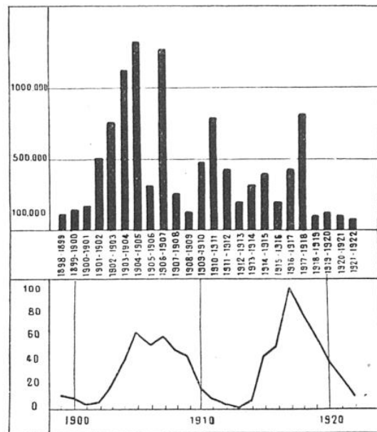
FIG. 14. — LE DIAGRAMME DE MORTALITÉ DE LA PESTE AUX INDES DE 1898 A 1922 (EN HAUT) SUIT L'ALLURE GÉNÉRALE DE LA COURBE DE L'ACTIVITÉ SOLAIRE
