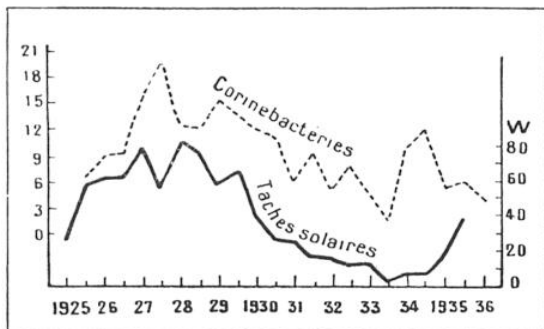
FIG. 6. — ACTIVITÉ SOLAIRE ET DÉVELOPPEMENT DE BACTÉRIES
