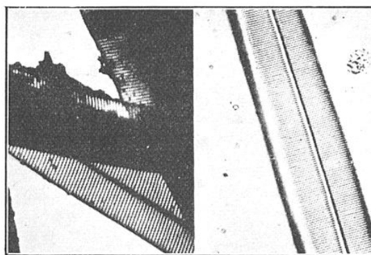
FIG. 9. — PHOTOGRAPHIES DE DIATOMÉES FORTEMENT AGRANDIES
