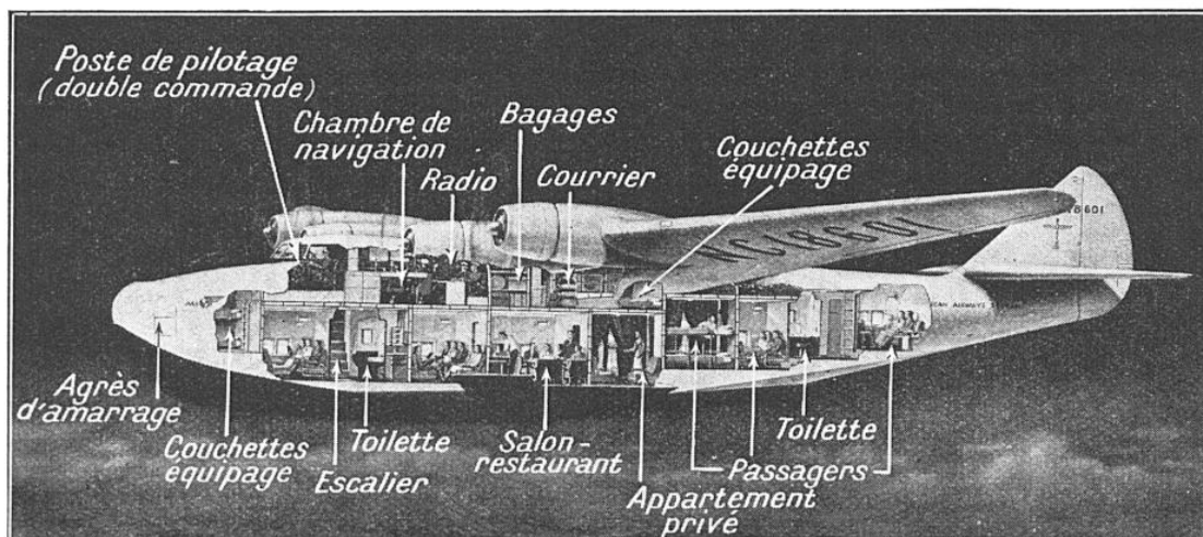
FIG. 10. — LES AMÉNAGEMENTS INTÉRIEURS DES HYDRAVIONS TRANSATLANTIQUES GÉANTS « BOEING 314 » EN ACHÈVEMENT EN AMÉRIQUE
