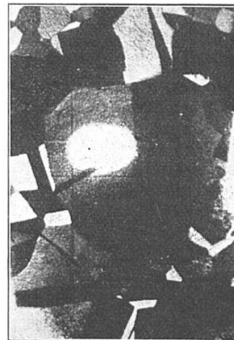
FIG. 6. — IMAGE ÉLECTRONIQUE D'UNE CATHODE INCANDESCENTE CRISTALLINE EN NICKEL (GROSSISSEMENT ENVIRON 50 FOIS)
