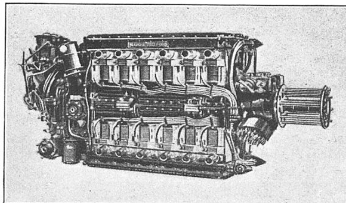
FIG. 7. — MOTEUR ANGLAIS « NAPIER-HALFORD DAGGER » DE 24 CYLINDRES EN H A REFROIDISSEMENT PAR AIR
