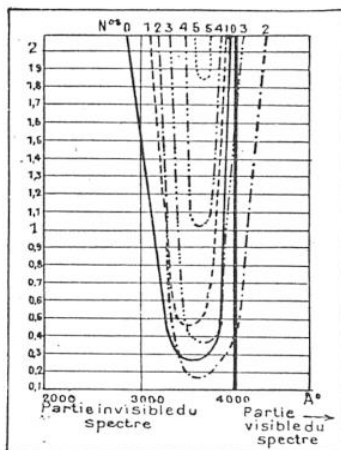
FIG. 5. — DIAGRAMMES DE DIVERS FILTRES PERMÉABLES AUX RAYONS ULTRAVIOLETS
