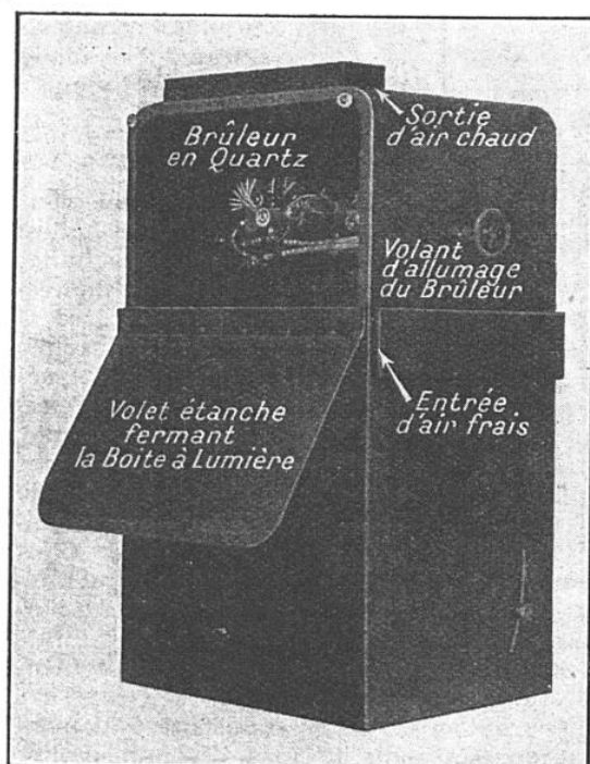
FIG. 6. — FACE ARRIÈRE D'UNE LANTERNE DE CONTROLE A LA LUMIERE DE WOOD, MONTRANT LE BRULEUR A VAPEUR DE MERCURE PRODUISANT LE RAYONNEMENT ULTRAVIOLET
