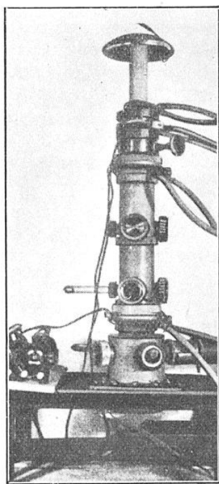
FIG. 8. — MICROSCOPE ÉLECTRONIQUE MAGNÉTIQUE CONSTRUIT SPÉCIALEMENT EN VUE DE L'OBTENTION DE TRÈS FORTS GROSSISSEMENTS (ENVIRON 10 000 FOIS)
