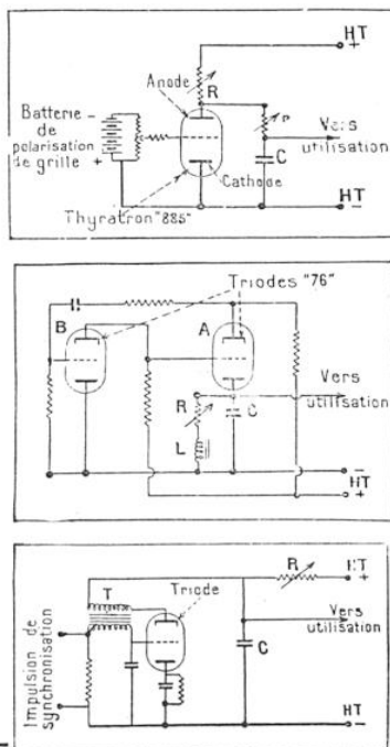
FIG. 1, 2, 3. — DISPOSITIFS FOURNISSENT DES TENSIONS EN « DENTS DE SCIE »
