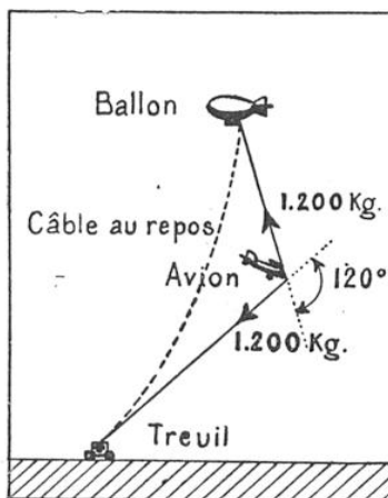
FIG. 4. — CAPTURE D'UN AVION PAR LE CÂBLE D'UN BALLON
