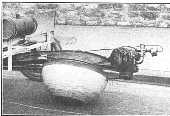
LA ROUE SPHÉRIQUE MOTRICE DU COLONEL LAMÉ DANS TROIS POSITIONS DIFFÉRENTES : EN HAUT, POSITION DISPOSÉE POUR LE MAXIMUM DE VITESSE (AXE HORIZONTAL) ; EN BAS, A GAUCHE, « POINT MORT » (AXE VERTICAL) ; A DROITE, POSITION INTERMÉDIAIRE (AXE INCLINÉ)
