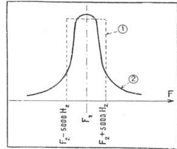
FIG. 6. — COURBES DE SÉLECTIVITÉ DE DEUX FILTRES DE BANDES, IDÉAL ET RÉEL
