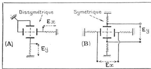
FIG. 4. — SCHÉMA DE PRINCIPE DE LA DÉFLEXION ELECTROSTATIQUE
