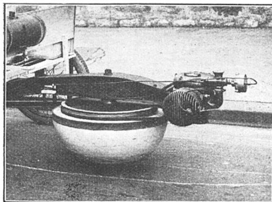
LA ROUE SPHÉRIQUE MOTRICE DU COLONEL LAMÉ DANS TROIS POSITIONS DIFFÉRENTES : EN HAUT, POSITION DISPOSÉE POUR LE MAXIMUM DE VITESSE (AXE HORIZONTAL) ; EN BAS, A GAUCHE, « POINT MORT » (AXE VERTICAL) ; A DROITE, POSITION INTERMÉDIAIRE (AXE INCLINÉ)
