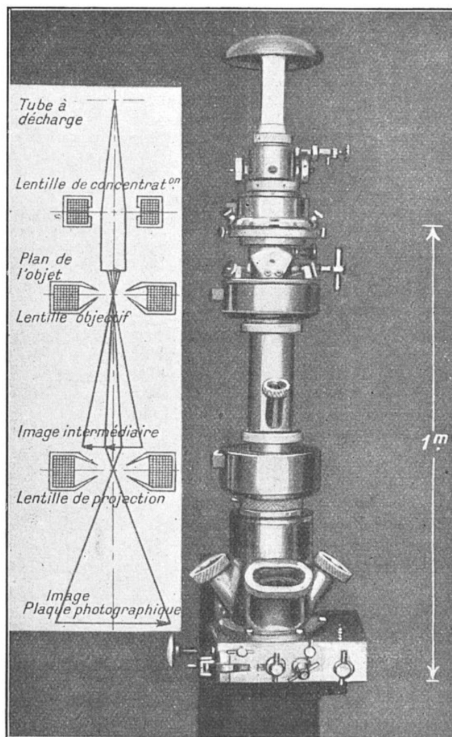
FIG. 12. — « SUPERMICROSCOPE » ÉLECTRONIQUE A COMMANDE MAGNÉTIQUE DE TRÈS HAUT RENDEMENT Le grossissement utile maximum de cet appareil atteint 20 000.
