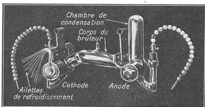
FIG. 2. — BRULEUR EN QUARTZ A VAPEUR DE MERCURE POUR LA PRODUCTION DE RAYONS ULTRAVIOLETS
