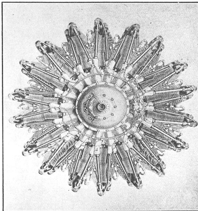
FIG. 3. — MOTEUR FRANÇAIS « GNOME ET RHONE L-18 » EN ÉTOILE A REFROIDISSEMENT PAR AIR
