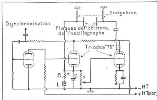
FIG. 5. — SYSTÈME DE DÉFLEXION SYMÉTRIQUE ÉQUIPÉ DE TRIODES A VIDE
