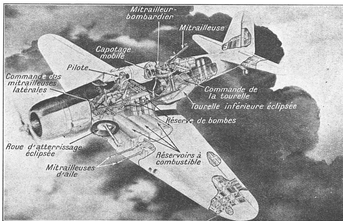
FIG. 9. — AVION DE COMBAT AMÉRICAIN « NORTHROP 8 A (A-17) »
