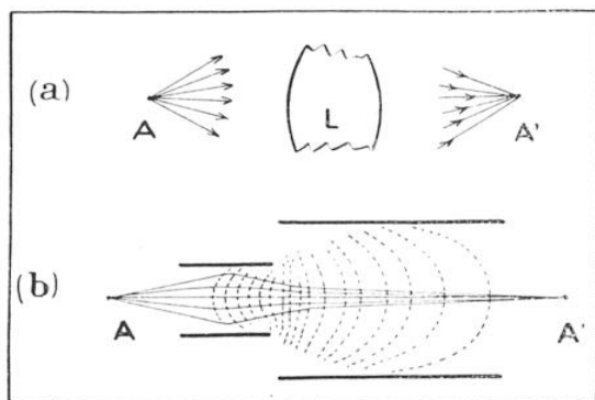
FIG. 2. — SCHÉMA DE PRINCIPE D'UNE LENTILLE ÉLECTRONIQUE
