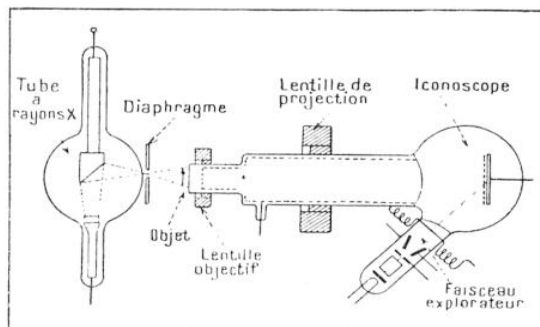
FIG. 7. — SCHÉMA D'UN MICROSCOPE ÉLECTRONIQUE MAGNÉTIQUE, MODIFIÉ D'APRÈS UN BREVET RÉCENT PRIS PAR LA MAISON ZEISS
