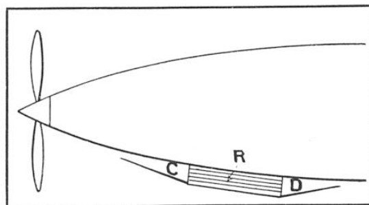
FIG. 2. — DISPOSITION SCHÉMATIQUE D'UN RADIATEUR « EN TUNNEL »
