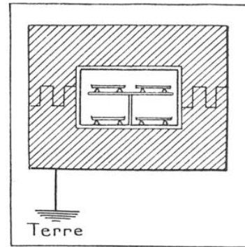
FIG. 4. — SCHÉMA DE L'INSTALLATION DESTINÉE À SOUS-TRAIRE DES CULTURES BIOLOGIQUES À L'ACTION DES RADIATIONS EXTÉRIEURES, RAYONS COSMIQUES EN PARTICULIER
