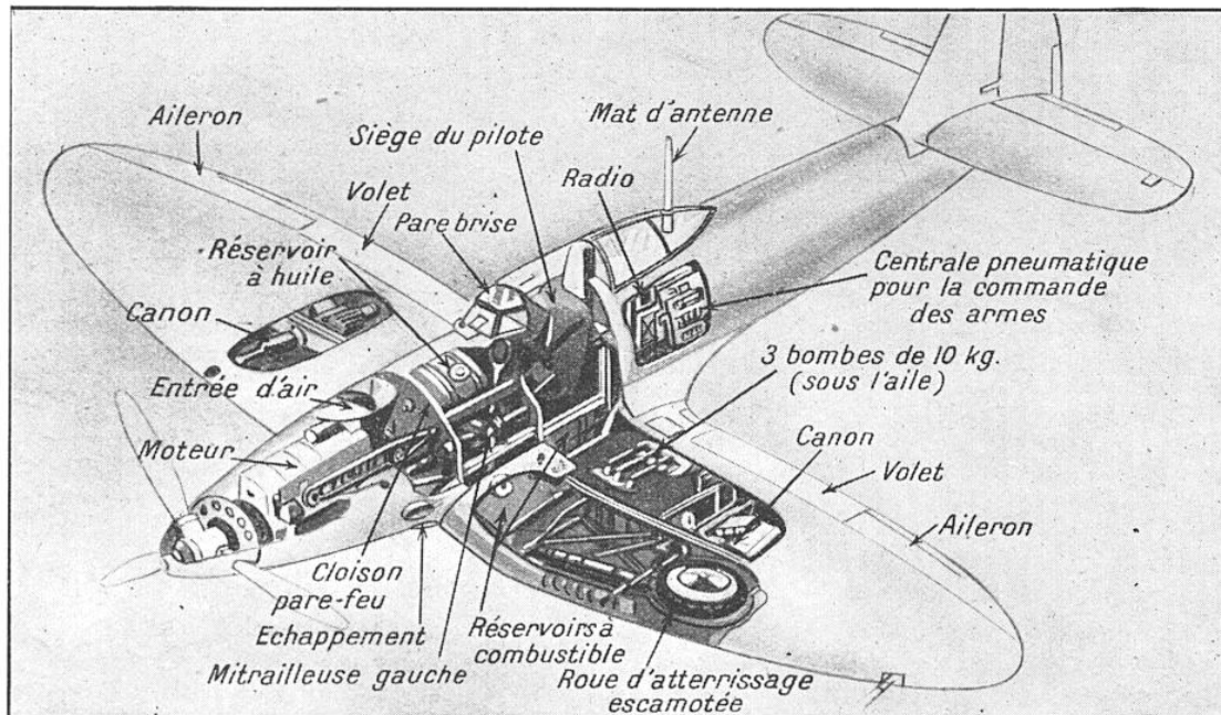
FIG. 1. — DÉTAIL DES AMÉNAGEMENTS DE L'AVION DE CHASSE ALLEMAND « HEINKEL-112 » C'est un monoplan à aile basse entièrement métallique de 9 m d'envergure, avec train d'atterrissage éclip-sable. Il est équipé d'un moteur à refroidissement par eau de 685 ch et sa vitesse maximum serait de 485 km/h. Il est armé de 2 mitrailleuses fixes sur les parois latérales du capot et de deux canons dans les ailes. Il emporte, en outre, 6 bombes légères.
