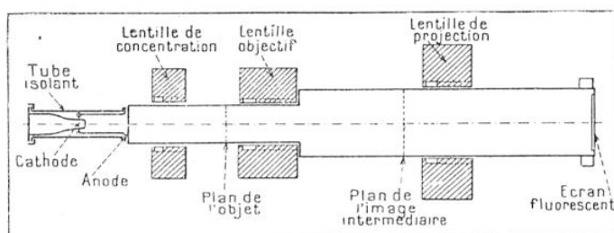
FIG. 3. — MICROSCOPE ÉLECTRONIQUE MAGNÉTIQUE
