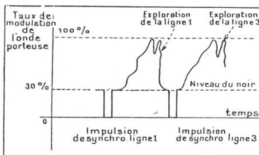
FIG. 6. — LES IMPULSIONS DE SYNCHRONISATION DE LIGNES SUPERPOSÉES A LA MODULATION DE L'ONDE PORTEUSE, DANS LES SYSTÈMES AUJOURD'HUI CLASSIQUES
