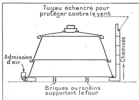
FIG. 2. — SCHÉMA D'UN FOUR MÉTALLIQUE COMPOSÉ D'ANNEAUX SUPERPOSÉS
