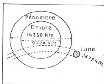
FIG. 2. — DIMENSIONS COMPARÉES DES SECTIONS DES CONES D'OMBRE ET DE PÉNOMBRE PROJETÉS PAR LA TERRE ET DU DIAMÈTRE DE LA LUNE
