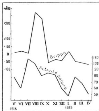
FIG. 13. — LA DIFFUSION DE LA GRIPPE DANS L'ARMÉE FRANÇAISE EN 1918-1919 APPARAÎT EN CORRÉLATION AVEC LES VARIATIONS DE L'ACTIVITÉ SOLAIRE PENDANT LA MÊME PÉRIODE
