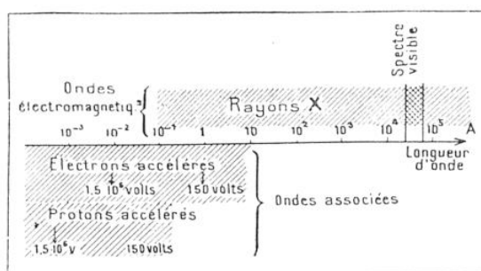
FIG. 1. — TABLEAU COMPARATIF DES LONGUEURS D'ONDE, DES ONDES ÉLECTROMAGNÉTIQUES ET DES ONDES ASSOCIÉES AUX CORPUSCULES, CALCULÉES D'APRÈS LA THÉORIE DE LA MÉCANIQUE ONDULATOIRE
