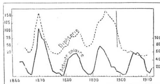
FIG. 15. — L'ACTIVITÉ SOLAIRE ET LA DIPHTÉRIE AU DANEMARK
