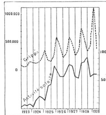
FIG. 7. — ACTIVITÉ SOLAIRE ET GRIPPE EN U. R. S. S. (DONNÉES TRIMESTRIELLES)
