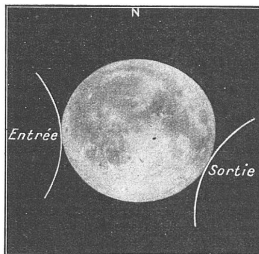
FIG. 3. — COMMENT SE PRÉSENTERA L'ÉCLIPSE DE LUNE DU 7 NOVEMBRE 1938
