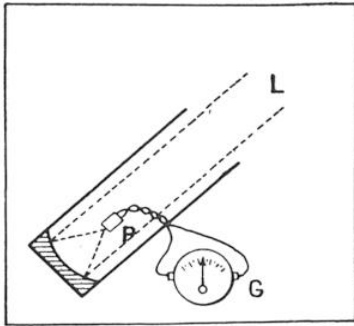
FIG. 5. — COMMENT ON MESURE LA TEMPÉRATURE D'UN ASTRE
