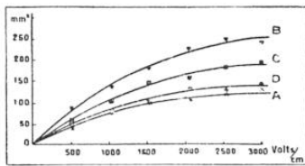
FIG. 5. — ACTION D'UN BOMBARDEMENT IONIQUE SUR UNE CULTURE DE STAPHYLOCOQUES
