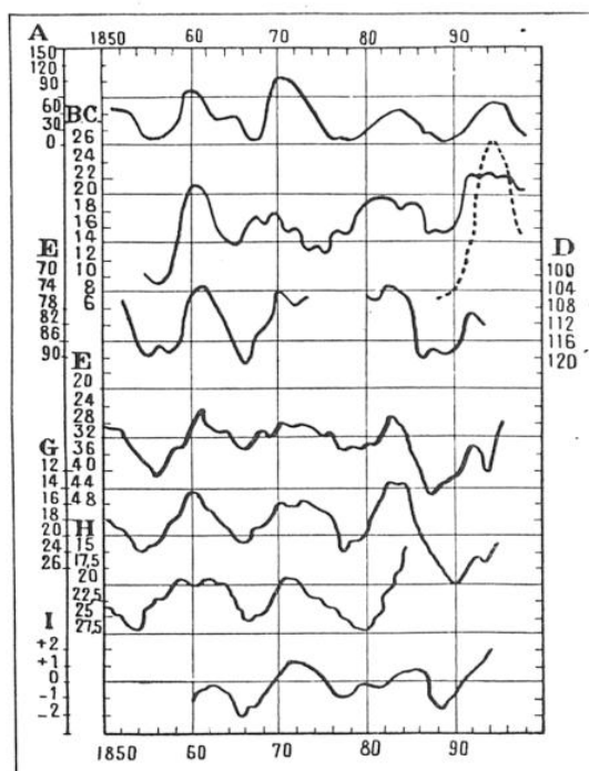
FIG. 11. — DE NOMBREUX PHÉNOMÈNES NATURELS SUIVENT LES VARIATIONS PÉRIODIQUES DE L'ACTIVITÉ SOLAIRE
