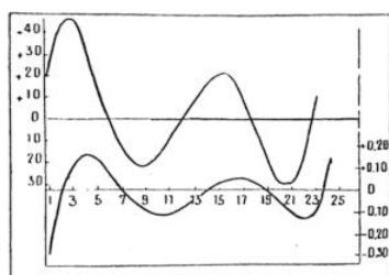
FIG. 9. — ACTIVITÉ SOLAIRE ET RÉCOLTES DE CÉRÉALES. Courbes montrant les oscillations moyennes, pendant un siècle d'observation, des récoltes de céréales en Russie (en bas) et du nombre des taches solaires (en haut).
