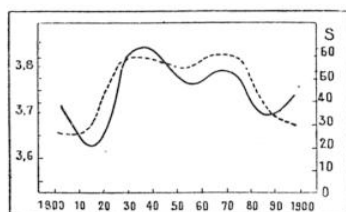
FIG. 10. — ACTIVITÉ SOLAIRE ET NATALITÉ EN EUROPE
