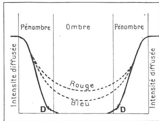
FIG. 7. — COURBES MONTRANT LES VARIATIONS DES ÉCLAIREMENTS DIFFUSÉS PAR LA LUNE AU COURS D'UNE ÉCLIPSE
