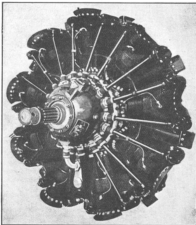
FIG. 6. — MOTEUR AMÉRICAIN « WRIGHT CYCLONE » EN ÉTOILE A REFROIDISSEMENT PAR AIR
