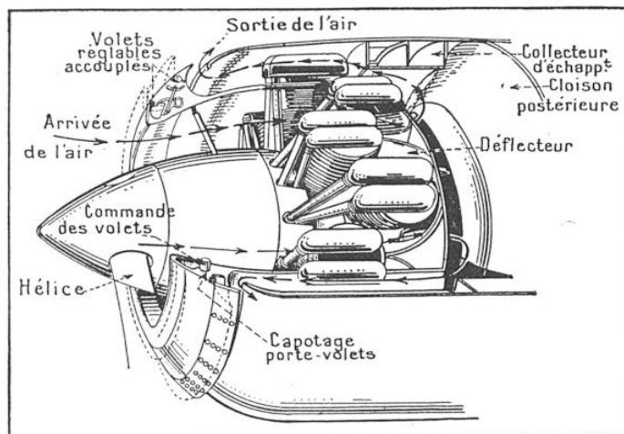
FIG. 1. — SCHÉMA DE LA CIRCULATION DE L'AIR DANS UN SYSTÈME NOUVEAU DE REFROIDISSEMENT PAR AIR POUR LES MOTEURS EN ÉTOILE
