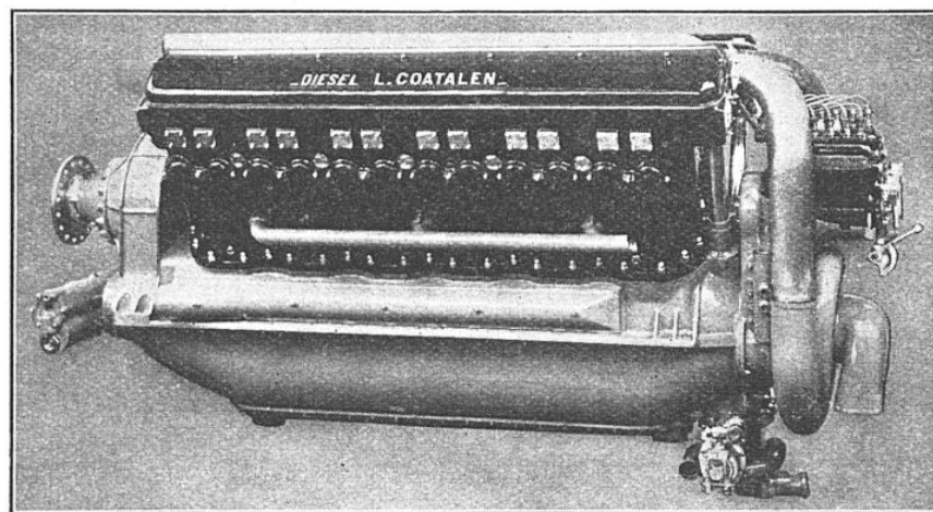
FIG. 8. — MOTEUR DIESEL D'AVIATION FRANÇAIS « COATALEN »
