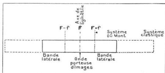
FIG. 1. — LA MODULATION DE L'ONDE PORTEUSE D'IMAGES DANS LE SYSTÈME DU MONT
