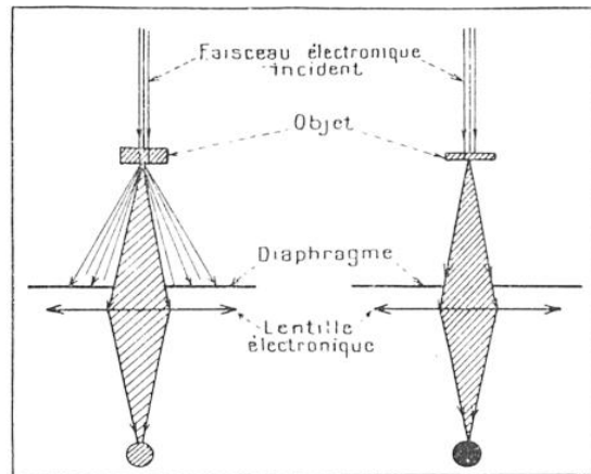
FIG. 5. — FORMATION DE L'IMAGE À TRAVERS UNE LENTILLE ÉLECTRONIQUE
