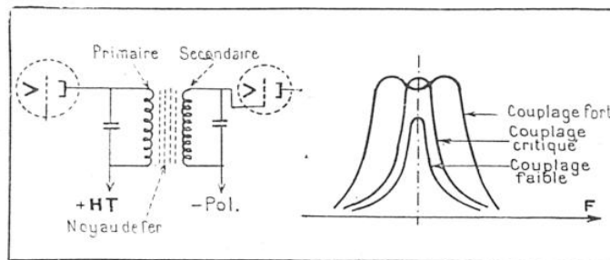
FIG. 7. — COURBES DE SÉLECTIVITÉ (À DROITE) DE DEUX CIRCUITS ACCORDÉS SUR LA MÊME FRÉQUENCE POUR DIFFÉRENTS COEFFICIENTS DE COUPLAGE (À GAUCHE)
