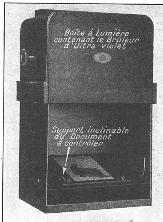
FIG. 7. — VOICI COMMENT ON DISPOSE LE DOCUMENT A CONTROLER A LA LUMIERE DE WOOD DANS LA LANTERNE DE LA FIGURE 6, VUE ICI SUR SA FACE AVANT
