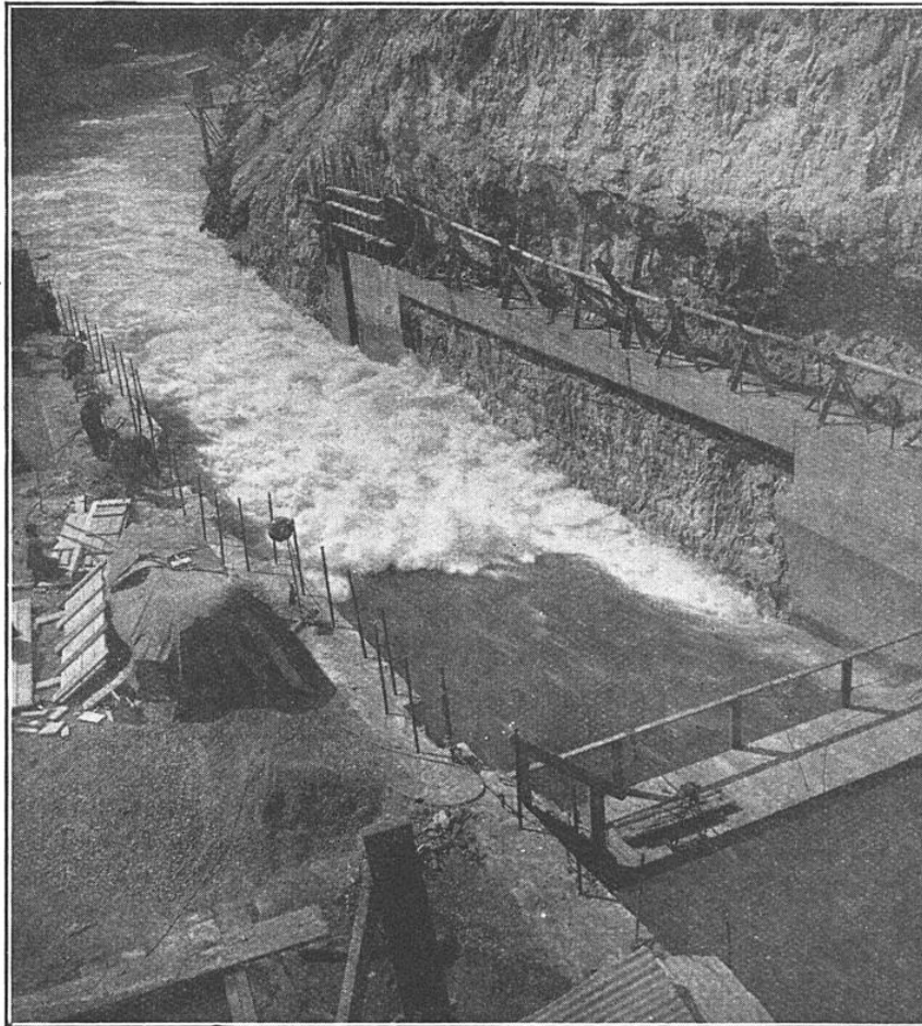
FIG. 8. — LE « RESSAUT » DU COURANT DE DÉRIVATION A LA SORTIE DU TUNNEL DE LA RIVE DROITE
