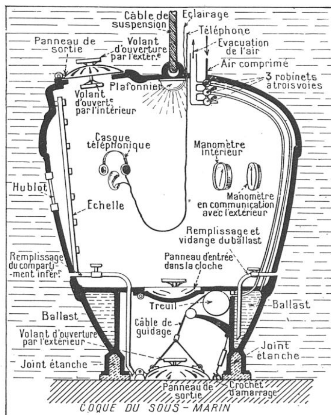
FIG. 7. — SCHÉMA DE PRINCIPE DE LA « CLOCHE »
