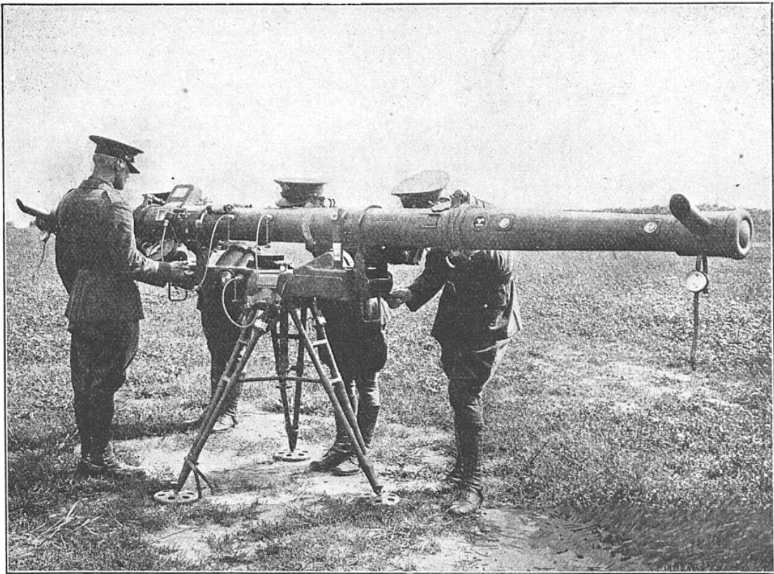
FIG. 9. — ALTI-TÉLÉMÈTRE POUR TIR CONTRE AVIONS
