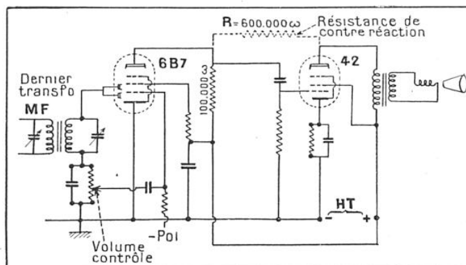
FIG. 5. — CONTRE-RÉACTION APPLIQUÉE AU DERNIER ÉTAGE D'UN AMPLIFICATEUR B. F. TRÈS CLASSIQUE
