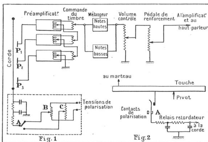
FIG. 1 ET 2. — SCHÉMA D'ENSEMBLE DU PIANO « ÉLECTRONIQUE » ET DÉTAIL DU DISPOSITIF DE COMMANDE DE LA POLARISATION DES CORDES POUR LE PASSAGE DU « PIANO » A L'« ORGUE » ET AU « BANJO »
