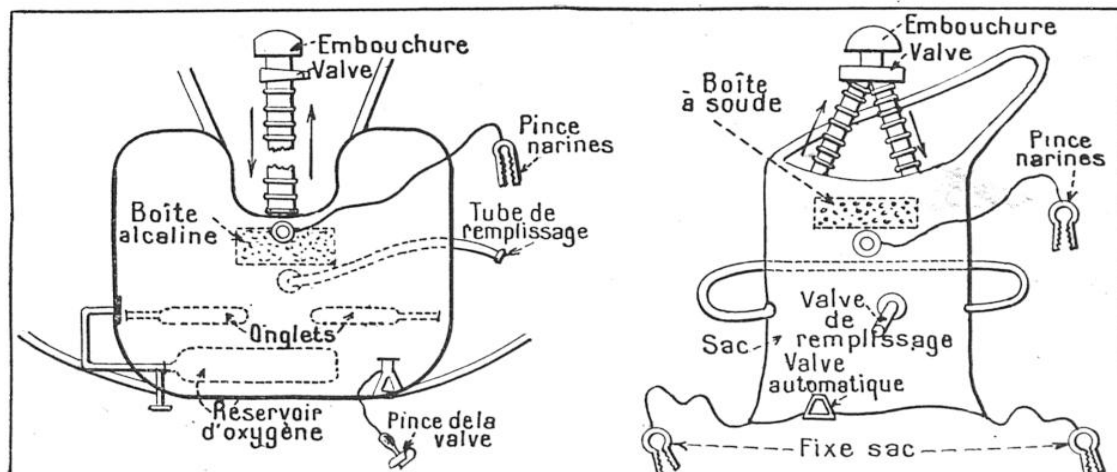
FIG. 4. — LES APPAREILS INDIVIDUELS « DAVIS » (ANGLAIS) ET « LUNG » (AMÉRICAIN)
