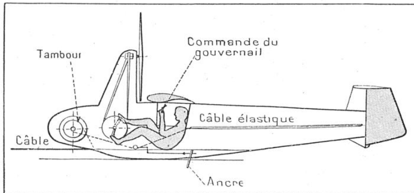
FIG. 4. — DISPOSITIFS DE PROPULSION, DE COMMANDE ET DE LANCEMENT DE L'APPAREIL HAESSLER ET VILLINGER
