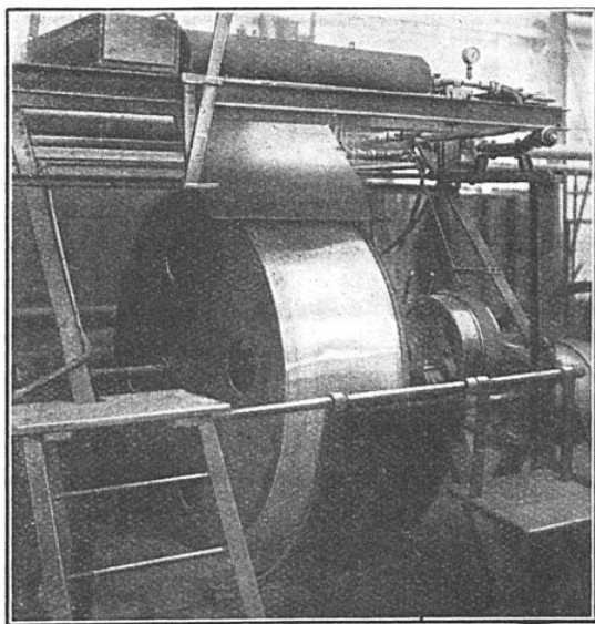
FIG. 1. — FABRICATION DE LA SOIE DE VERRE
