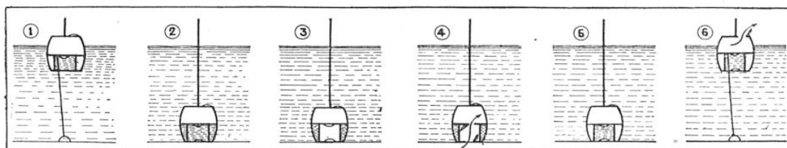
FIG. 8. — PRINCIPE DES MANŒUVRES SUCCESSIVES POUR LE SAUVETAGE PAR LA « CLOCHE »
