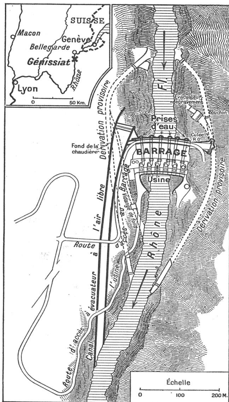
FIG. 1. — PLAN GÉNÉRAL DE L'USINE FUTURE
