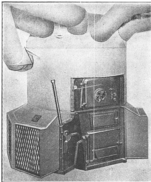
FIG. 7. — FILTRE « DUSTOP » EN FIBRES DE VERRE, SUR UNE CHAUDIÈRE DE CALORIFÈRE
