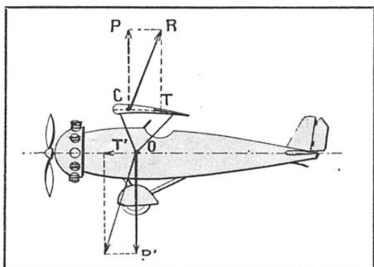
FIG. 1. — PRINCIPE DE LA SUSTENTATION D'UN AVION EN VOL
