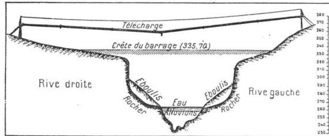
FIG. 3. — COUPE TRANSVERSALE DU SITE DE GÉNISSIA. Elle montre les profils du lit rocheux, du lit alluvionnaire et des éboulis, qui sont les premiers facteurs naturels dont les ingénieurs ont eu à traiter pour établir leur devis.
