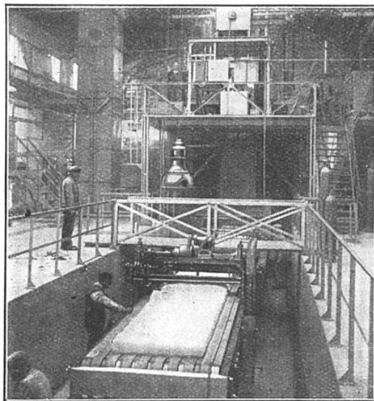
FIG. 2. — ENSEMBLE D'UNE INSTALLATION DE FABRICATION DE LAINE DE VERRE
