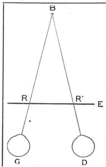
FIG. 1. — MESURE DE LA PARALLAXE D'UN BUT Sur l'écran transparent E, placé à une distance connue des yeux, on marque R et R' à l'intersection des rayons GB et DB. On peut ainsi construire le trapèze GRR'D et, par conséquent, la parallaxe GBD du point B.
