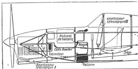
FIG. 6. — DISPOSITIF DE MANŒUVRE DE L'EXTINCTEUR ET DE RUPTURE DU CONTACT D'ALLUMAGE ET DES CIRCUITS ÉLECTRIQUES
