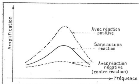
FIG. 1. — INFLUENCE DES RÉACTIONS POSITIVES ET NÉGATIVES SUR LA « COURBE DE RÉPONSE » D'UN AMPLIFICATEUR BASSE FRÉQUENCE
