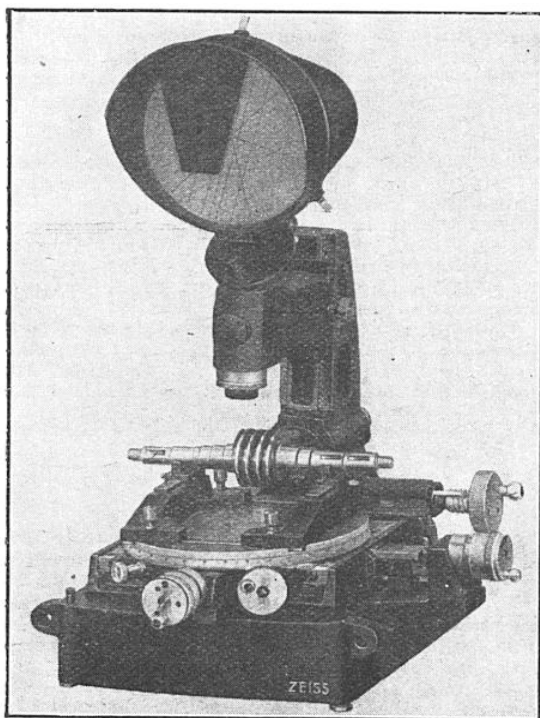
FIG. 7. — VÉRIFICATION D'UNE VIS SANS FIN On voit sur l'écran supérieur le profil du filet de la vis en même temps que les lignes de repère qui sont la projection des réticules de l'oculaire.
