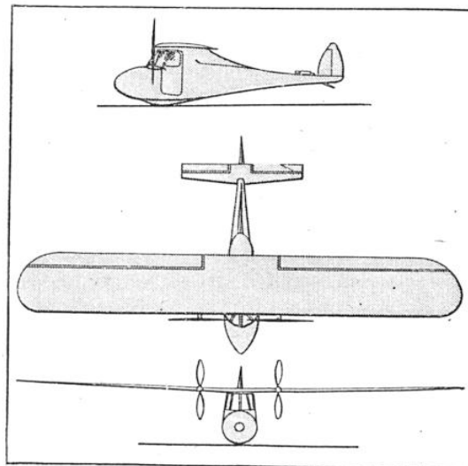
FIG. 2. — L'AVION BOSSI-BONOMI A PROPULSION MUSCULAIRE
