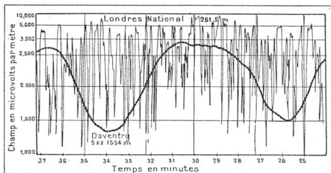
FIG. 8. — COMMENT VARIE L'ÉVANOUISSEMENT DES ONDES OU FADING
