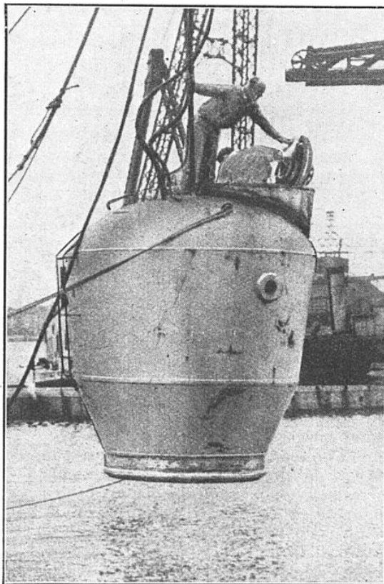
FIG. 6. — LA « CLOCHE » SOUS-MARINE UTILISÉE POUR LE SAUVETAGE DU « SQUALUS »
