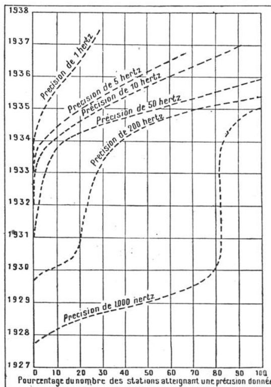
FIG. 2. — AMÉLIORATION PROGRESSIVE DE LA STABILITÉ DES CENT MEILLEURS ÉMETTEURS EUROPÉENS
