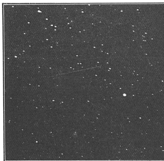
FIG. 4. — LA PETITE PLANÈTE HERMÈS, QUI RASA LA TERRE LE 30 OCTOBRE 1937
