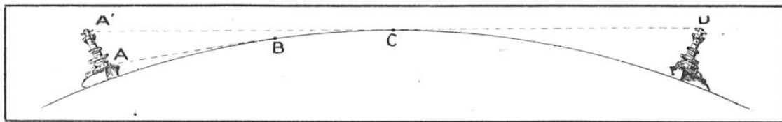
FIG. 8. — L'HORIZON EST LIMITÉ PAR LA COURBURE TERRESTRE
