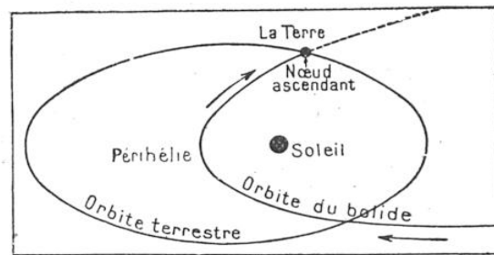
FIG. 6. — L'ORBITE PROBABLE DE LA GRANDE MÉTÉORITE DE SIBÉRIE
