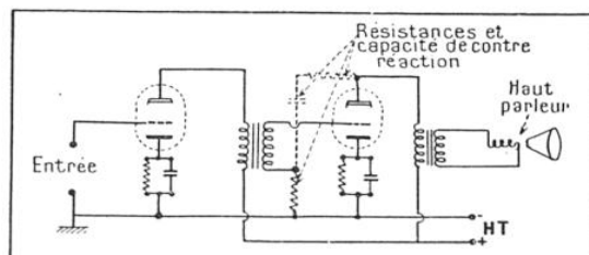
FIG. 4. — CONTRE-RÉACTION APPLIQUÉE AU DERNIER ÉTAGE D'UN AMPLIFICATEUR B. F.
