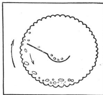
FIG. 6. — SCHÉMA DU TRIEUR ROTATIF
