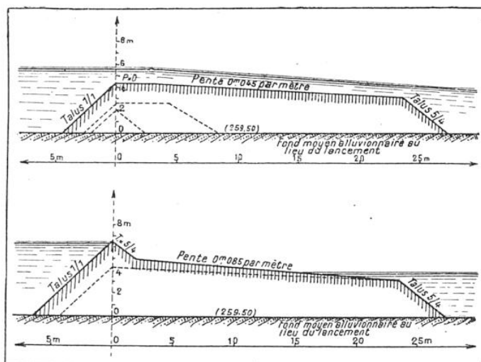
FIG. 5. — LES PHASES DE LA « COUPURE » DU FLEUVE, SUIVANT L'APPLICATION DU SYSTÈME ISBACH
