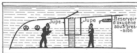
FIG. 2. — LA « JUPE » DANS UN SOUS-MARIN
