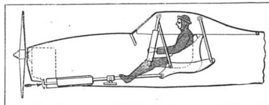
FIG. 4 ET 5. — POSITIONS DU SIÈGE ET DU PILOTE AVANT ET APRÈS LE CONTACT BRUSQUE DE L'AVION AVEC LE SOL
