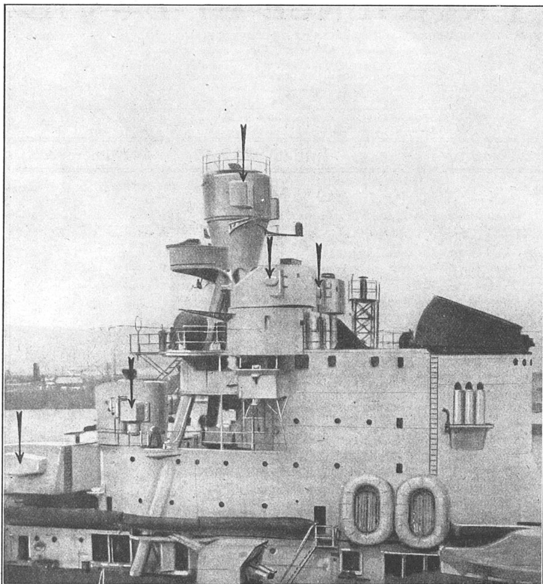
LES CINQ TOURELLES DE TÉLÉMÉTRIE (INDIQUÉES PAR DES FLÈCHES) INSTALLÉES SUR LA MÂTURE AVANT D'UN DES DERNIERS CROISEURS ITALIENS DE 10 000 T, LE « POLA »
