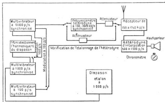
FIG. 4. — SCHÉMA DE PRINCIPE DU DISPOSITIF DE MESURE POUR LES FRÉQUENCES MOYENNES DE LA BANDE DE 150 A 1 750 KILOHERTZ
