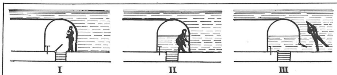
FIG. 1. — PRINCIPE DE FONCTIONNEMENT D'UN « SAS » DE SORTIE
