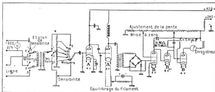
FIG. 6. — SCHÉMA DU MODULOMÈTRE SERVANT À LA MESURE DU TAUX DE MODULATION DES ÉMISSIONS
