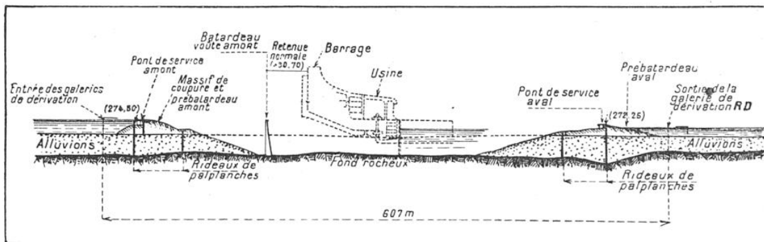
FIG. 4. — COUPE LONGITUDINALE DU SITE DE GÉNISSIA
