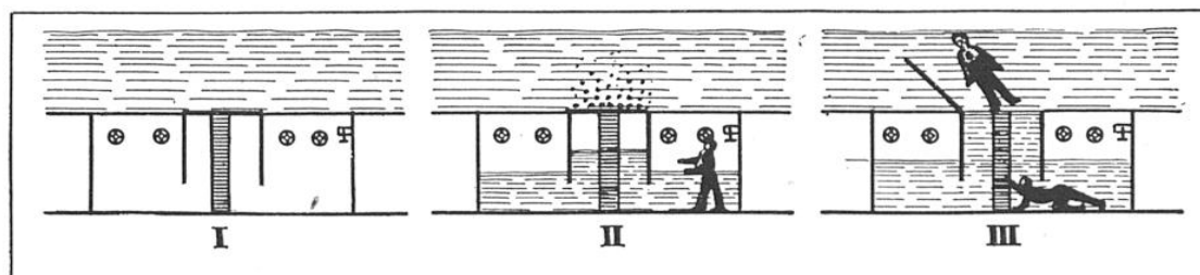
FIG. 3. — PRINCIPE DE LA MANŒUVRE DE SORTIE A L'AIDE DE LA « JUPE »
