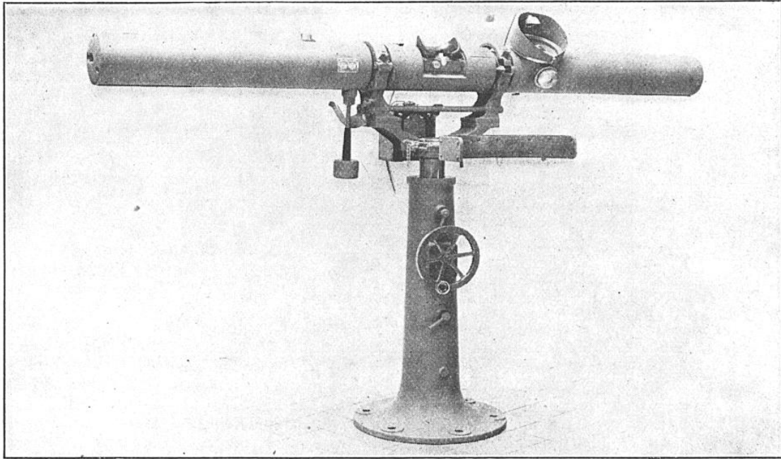
FIG. 6. — TÉLÉMÈTRE STÉRÉOSCOPIQUE DE 2 M DE BASE UTILISÉ A BORD DU « NORMANDIE » Il permet de repérer les bouées ou balises jusqu'à 5 à 6 km avec une erreur qui n'est pas supérieure à 200 m
