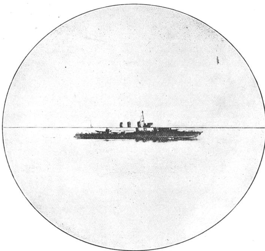
FIG. 2. — ASPECT DU CHAMP D'UN TÉLÉMÈTRE À COÏNCIDENCE La partie supérieure de l'image est décalée vers la gauche ; la mise en coïncidence des cheminées et des mâts permet de mesurer la distance du bâtiment.
