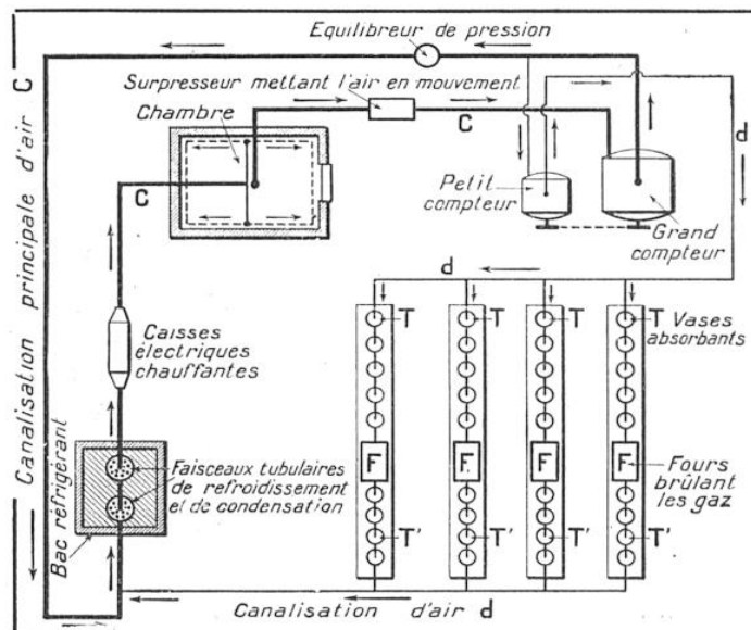
FIG. 3. — SCHÉMA GÉNÉRAL DU LABORATOIRE DE BIO-ÉNERGÉTIQUE DE M. LEFÈVRE
