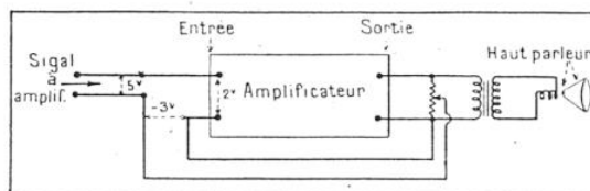
FIG. 2. — PRINCIPE DE LA CONTRE-RÉACTION
