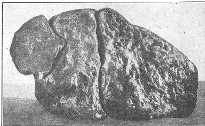
FIG. 9. — PHOTOGRAPHIE DE LA MÉTÉORITE D'UNE MASSE DE 234 KG TOMBÉE EN HONGRIE EN 1866
