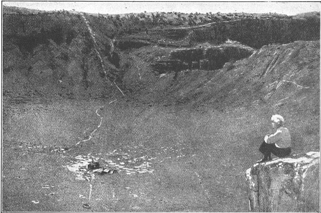
FIG. 8. — VUE DE L'INTÉRIEUR DU « METEOR CRATER »
