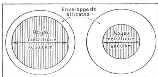
FIG. 5. - LA STRUCTURE INTERNE DE LA TERRE A droite, la Terre selon la conception courante : un noyau de ferro-nickel de 6 800 km de diamètre couvert d'une épaisse couche de silicates. A gauche, la Terre suivant le schéma de M. Dauvillier. Le globe n'est qu'une énorme météorite de ferro-nickel, qu'enveloppe une mince scorie de silicates.
