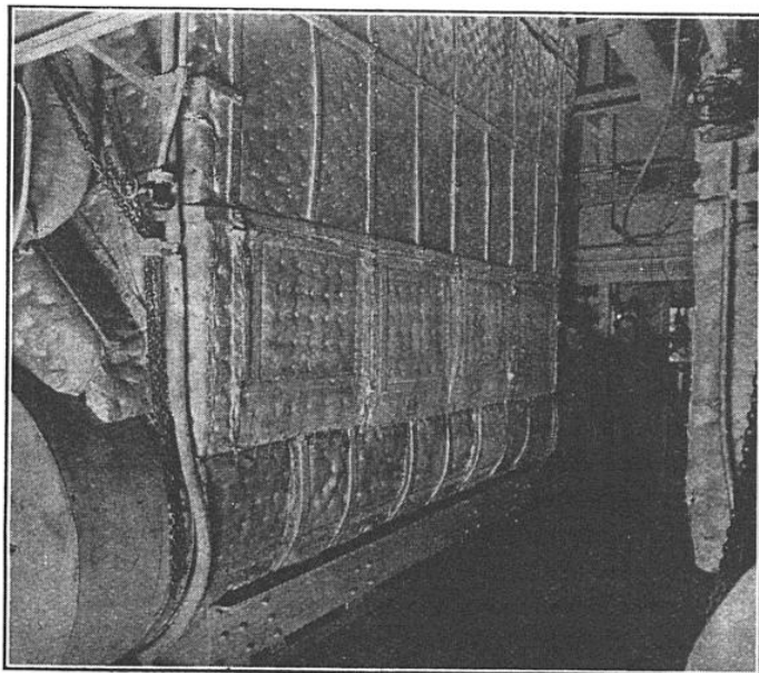
FIG. 5. — REVÊTEMENT D'UNE PAROI DE CHAUDIÈRE AVEC DES MATELAS DE SOIE DE VERRE
