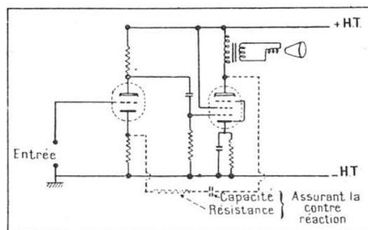
FIG. 3. — CONTRE-RÉACTION APPLIQUÉE AUX DEUX ÉTAGES D'UN AMPLIFICATEUR B. F.
