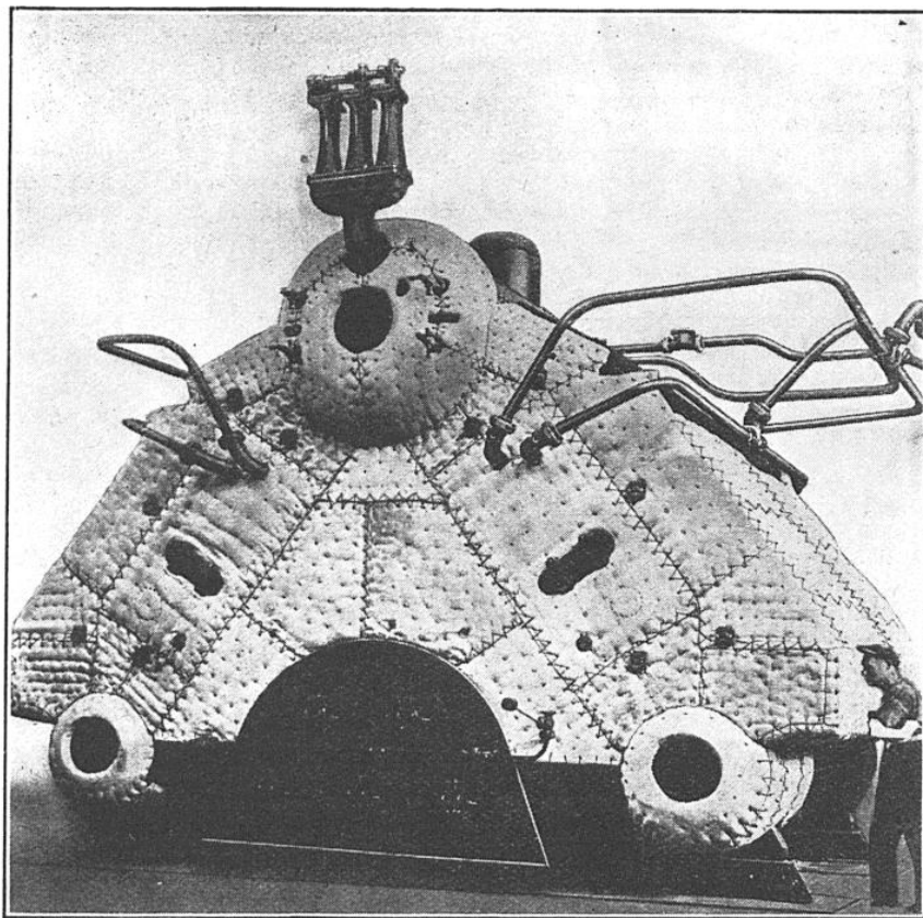
FIG. 4. — CALORIFUGEAGE D'UNE CHAUDIÈRE MARINE
