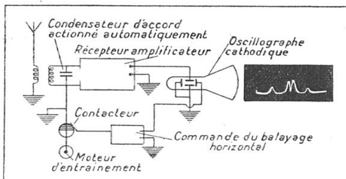
FIG. 6. — PRINCIPE DE L'APPAREIL DE GUIDAGE « PANORAMIQUE »
