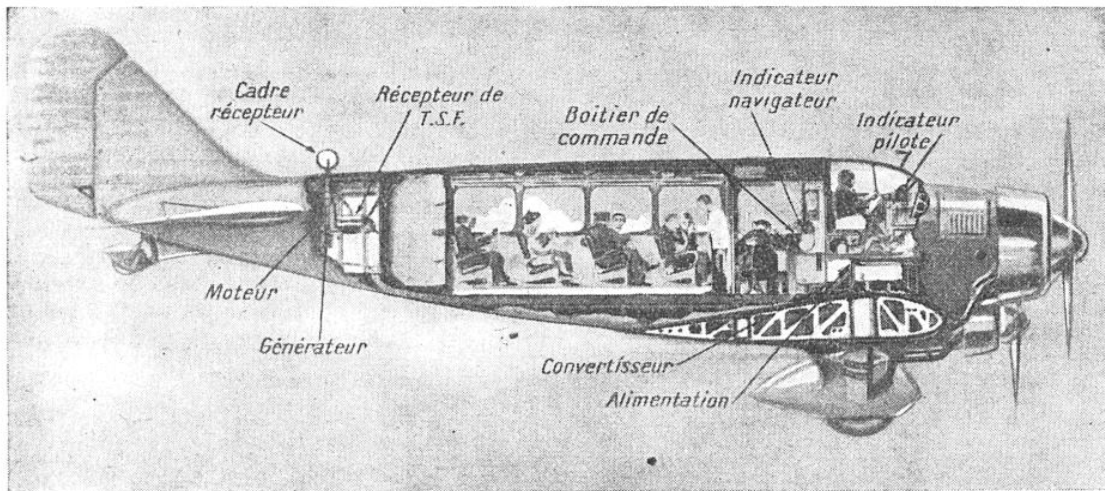
FIG. 4. — MONTAGE DU RADIOCOMPAS AUTOMATIQUE L. M. T. RC5 SUR UN AVION COMMERCIAL. Le cadre tournant est entraîné par le moteur-générateur, et connecté au récepteur de T. S. F.; son fonctionnement est contrôlé à distance par un boîtier de commande; l'alimentation est assurée par un convertisseur. Un « indicateur-navigateur » se trouve dans la cabine du navigateur et un « indicateur-pilote » dans celle du pilote.
