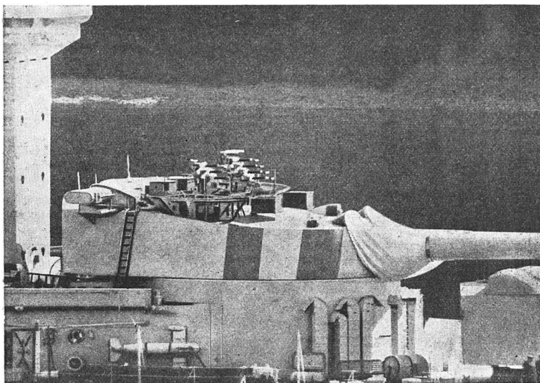
IG. 2. — DEUX AFFÛTS DE MITRAILLEUSES QUADRUPLES MONTÉS SUR LE TOIT DE LA TOURELLE AVANT SUPÉRIEURE D'UN CUIRASSÉ BRITANNIQUE (WARSPITE)
