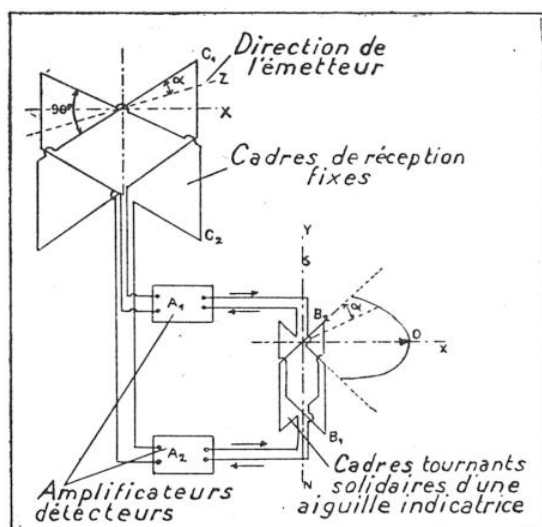
FIG. 2. — PRINCIPE DE LA BOUSSOLE HERTZIENNE
