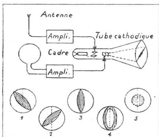
FIG. 5. — EMPLOI DE L'OSCILLOGRAPHIE CATHODIQUE COMME INDICATEUR VISUEL D'ORIENTATION
