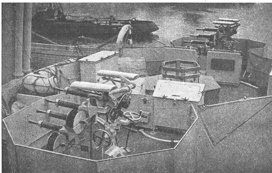
FIG. 6. — DEUX GROUPES DE MITRAILLEUSES DE 13 MM SUR LA PASSERELLE ARRIÈRE D'UN ESCORTEUR ANTIAÉRIEN BRITANNIQUE, TYPE « WHITLEY »
