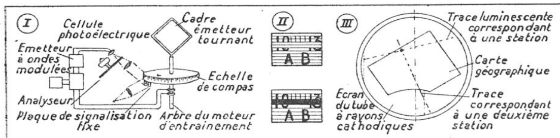
FIG. 8 — LE GUIDAGE DES AVIONS PAR TÉLÉVISION
