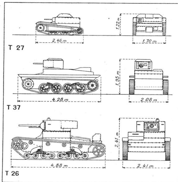
FIG. 1. — SCHEMAS DE PROFIL ET DE FACE DES CHARS DE RECONNAISSANCE ET CHARS LÉGERS DE L'ARMÉE ROUGE Voir les caractéristiques dans le texte (p 32).
