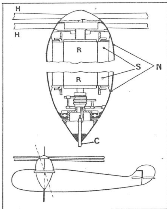
FIG. 1. — L'APPAREIL ANGLAIS POUR REMPLACER LES BALLONS A CABLES
