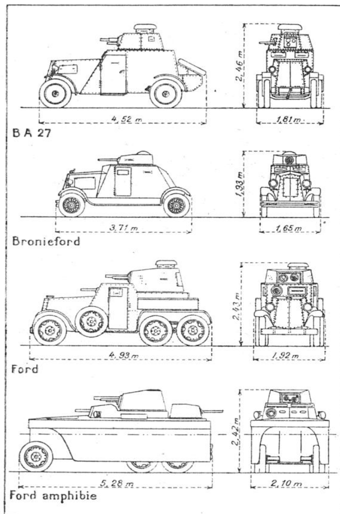
FIG. 3. — SCHÉMAS DE PROFIL ET DE FACE DES QUATRE MODÈLES D'AUTOMITRAILLEUSES EN SERVICE DANS LES GROUPES DE RECONNAISSANCE DE L'ARMÉE ROUGE
