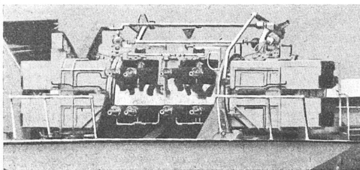
FIG. 1. — GROUPE DE CANONS « POM-POM » DE 40 MM VICKERS, SUR AFFÛT OCTUPLE, A BORD D'UN CROISIER ANTIAÉRIEN BRITANNIQUE
