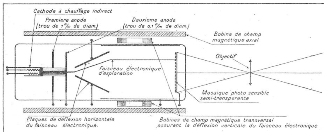
FIG. 1. — DISPOSITION DE PRINCIPE DES ÉLECTRODES DU NOUVEL ANALYSEUR ÉLECTRONIQUE DÉRIVÉ DE L'ICONOSCOPE : L'ORTHICON
