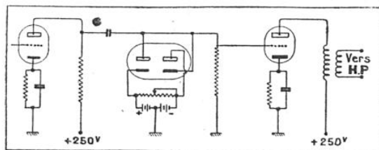
FIG. 1. — CIRCUIT LIMITEUR D'AMPLITUDE DESTINÉ A RABOTER TOUS LES PARASITES D'AMPLITUDE ÉLEVÉE
