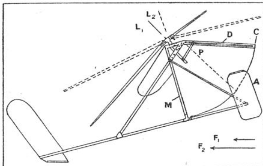
FIG. 2. — LE CERF-VOLANT AUTOGIRE AMÉRICAIN
