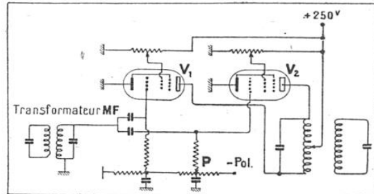
FIG. 2. — CIRCUIT DIFFÉRENTIEL LIMITEUR DE PARASITES
