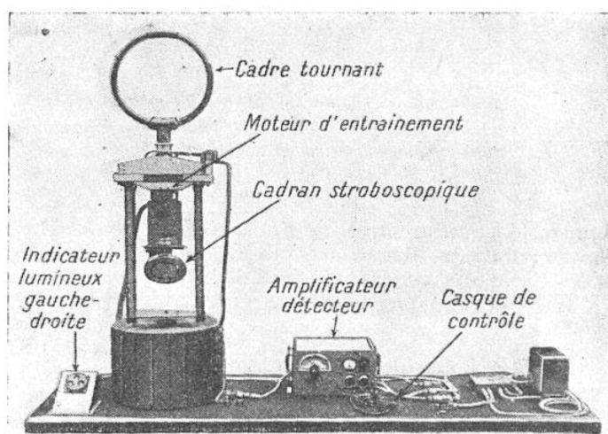
FIG. 3. — RADIOCOMPAS STROBOSCOPIQUE LEPAUTE A CADRE TOURNANT
