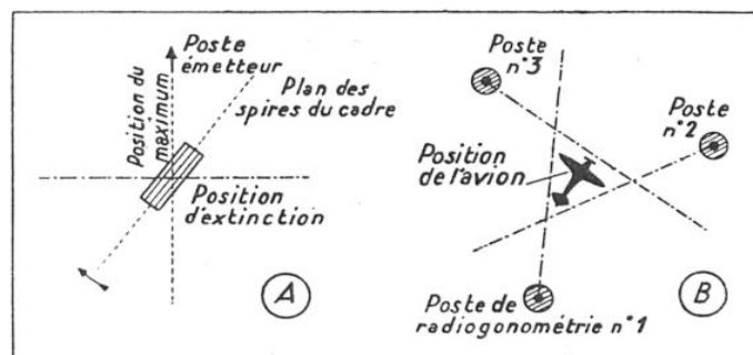
FIG. 1. — LE RELÈVEMENT D'UN AVION PAR LA RADIOGONIOMÉTRIE
