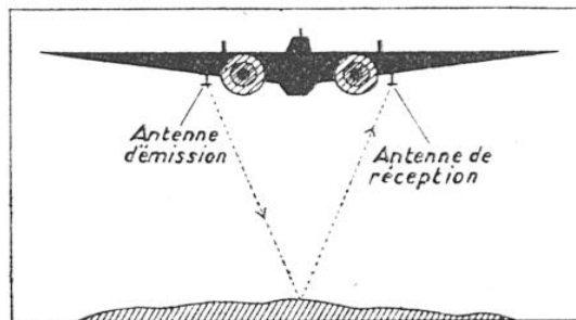
FIG. 7. — L'ALTIMÈTRE RADIOÉLECTRIQUE FONCTIONNANT PAR RÉFLEXION D'UN FAISCEAU D'ONDES ULTRA-COURTES SUR LA SURFACE DU SOL
