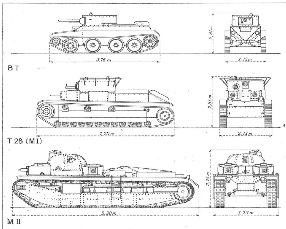
FIG. 6. — SCHÉMAS DE PROFIL ET DE FACE DES CHARS MOYENS ET LOURDS DE L'U. R. S. S.
