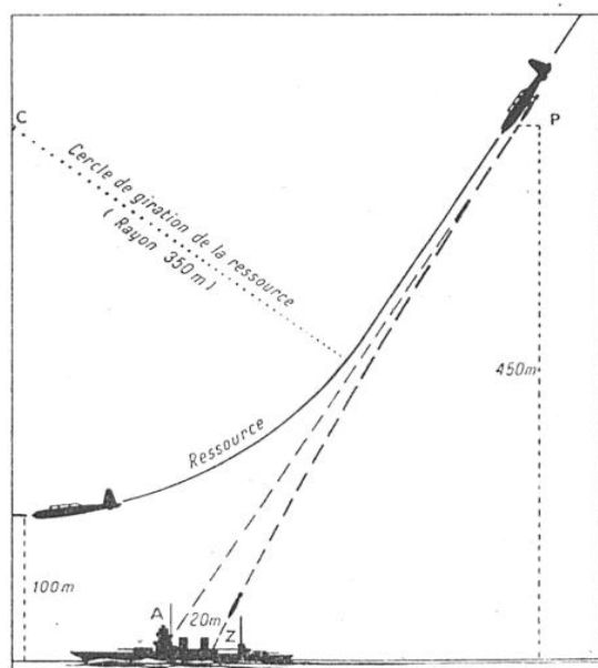
FIG. 6. — UN MORTIER LANCE-BOMBES PEUT-IL AMÉLIORER LE LANCEMENT EN PIQUÉ ?
