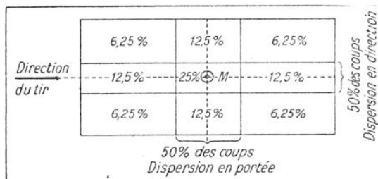
FIG. 6. — LA DISPERSION, CAUSE PRINCIPALE DU FAIBLE RENDEMENT DES PIÈCES D'ARTILLERIE
