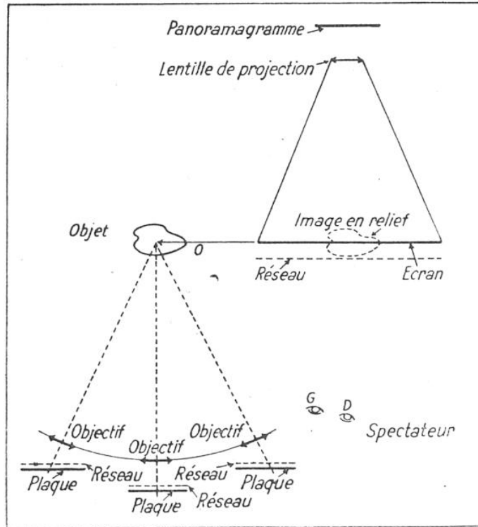
FIG. 8. — SCHÉMA DE PRINCIPE DE LA RÉALISATION ET DE L'UTILISATION D'UN PANORAMAGRAMME
