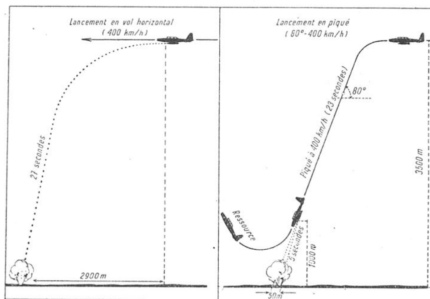
FIG. 1. — LANCEMENT EN VOL HORIZONTAL ET LANCEMENT EN PIQUÉ
