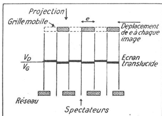
FIG. 5. — LA PROJECTION CINÉMATOGRAPHIQUE EN RELIEF A DEUX IMAGES
