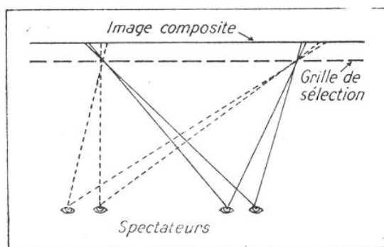
FIG. 6. — PRINCIPE DU PANORAMAGRAMME
