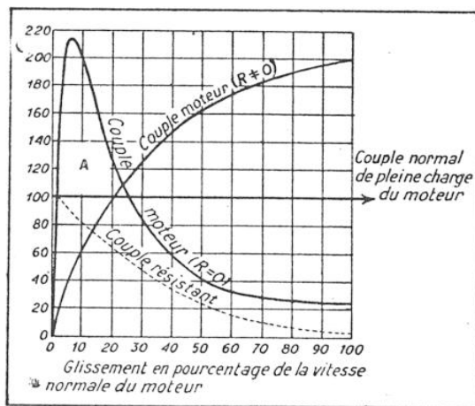
FIG. 3. — COURBE DONNANT LE COUPLE TRANSMIS EN FONCTION DU GLISSEMENT
