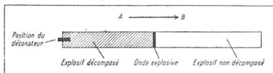
FIG. 6. — COMMENT SE PROPAGE L'ONDE EXPLOSIVE AU COURS D'UNE DÉTONATION
