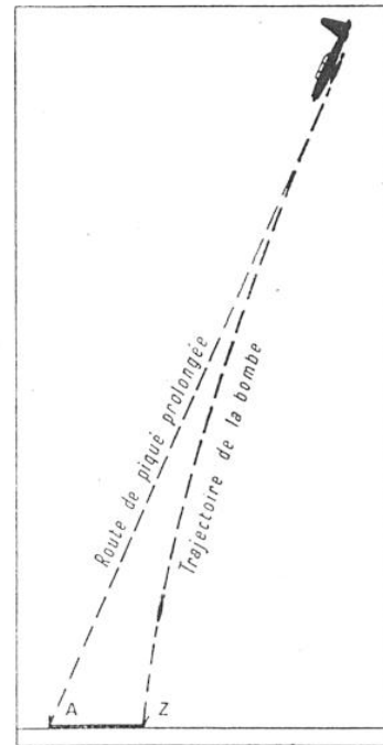
FIG. 5. — ÉCART EN PORTÉE DANS LE LANCEMENT EN SEMI-PIQUÉ
