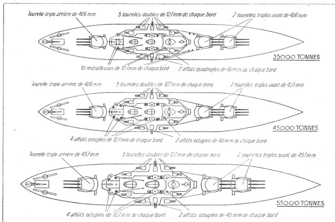
FIG. 1. — SCHÉMA DES NAVIRES DÉRIVÉS DU « NORTH CAROLINA »
