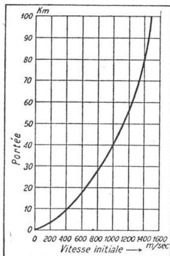
FIG. 1. — LA PORTÉE D'UNE BOUCHE À FEU AUGMENTE AVEC LA VITESSE INITIALE
