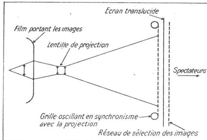
FIG. 9. — LA PROJECTION D'UNE IMAGE COMPOSITE POUR LE PANORAMAGRAMME ANIMÉ
