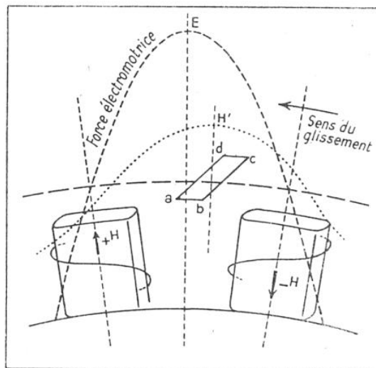
FIG. 2. — PRINCIPE DE FONCTIONNEMENT D'UN ACCOUPLEMENT ÉLECTROMAGNÉTIQUE ASYNCHRONE
