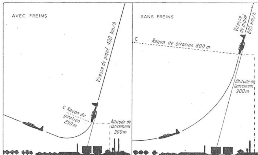
FIG. 2. -- LES FREINS DE PIQUÉ PERMETTENT UN LANCEMENT A PLUS FAIBLE ALTITUDE, DONC PLUS PRÉCIS
