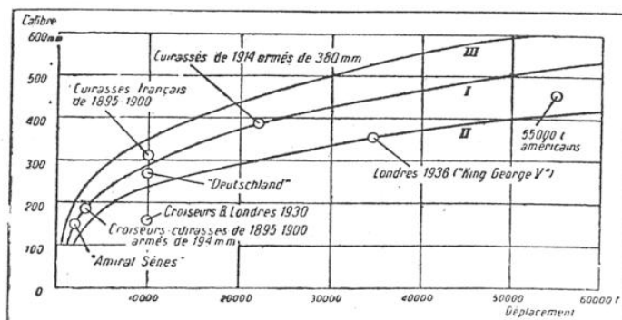
FIG. 4. — LOIS DE CROISSANCE DU CALIBRE DE L'ARTILLERIE AVEC LE DÉPLACEMENT DES NAVIRES DE GUERRE
