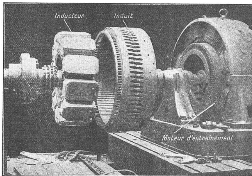
FIG. 4. — ACCOUPLEMENT ÉLECTROMAGNÉTIQUE A GLISSEMENT EN COURS D'ESSAIS, MONTRANT LES DEUX PARTIES TOURNANTES SÉPARÉES
