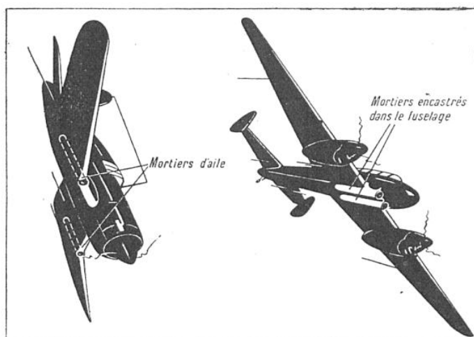
FIG. 7. — DEUX DISPOSITIONS POSSIBLES POUR DES MORTIERS LANCE-BOMBES A BORD D'UN AVION
