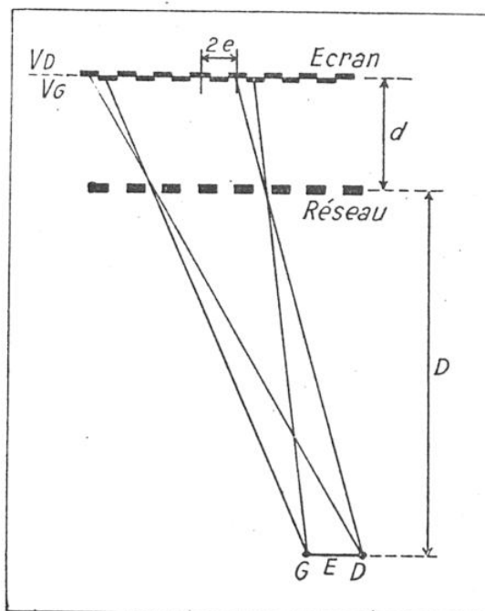
FIG. 4. — LA SÉPARATION DES IMAGES PAR LE PROCÉDÉ DES RÉSEAUX
