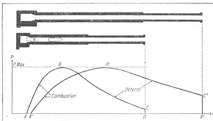
FIG. 3. — LA RECHERCHE DU MEILLEUR RENDEMENT BALISTIQUE D'UNE BOUCHE À FEU
