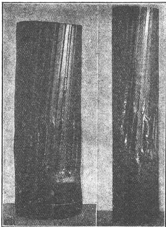
FIG. 4. — DEUX STADES DIFFÉRENTS DE L'USURE D'UNE BOUCHE A FEU
