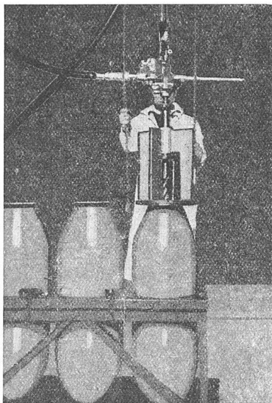
FIG. 5. — PERCEUSE PNEUMATIQUE CREUSANT DANS L'EXPLOSIF D'UNE BOMBE LE LOGEMENT D'UN RELAIS DE TÉTRYL
