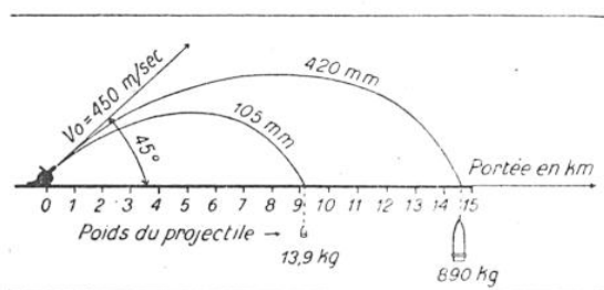
FIG. 2. — LA PORTÉE DES PIÈCES D'ARTILLERIE CROÎT AVEC LE POIDS DU PROJECTILE
