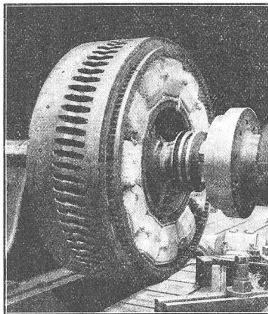
FIG. 1. — UN ACCOUPLEMENT ÉLECTROMAGNÉTIQUE POUR REMORQUEUR
