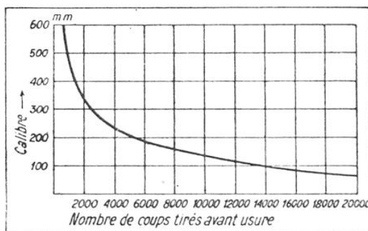
FIG. 5. — LA LONGÉVITÉ D'UNE BOUCHE A FEU DÉCROÎT RAPIDEMENT QUAND SA PUISSANCE AUGMENTE
