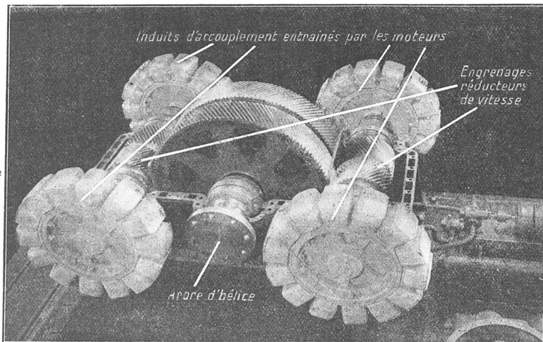
FIG. 5. — VUE EN BOUT D'UN RÉDUCTEUR DE VITESSE A ENGRENAGES AVEC LES TÊTES D'INDUIT DES ACCOUPLEMENTS ÉLECTROMAGNÉTIQUES POUR QUATRE MOTEURS DIESEL DE 1 100 CH CHACUN
