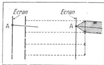
FIG. 10. — UN ÉCRAN SÉLECTEUR FORMÉ DE PRISMES CONVERGENTS
