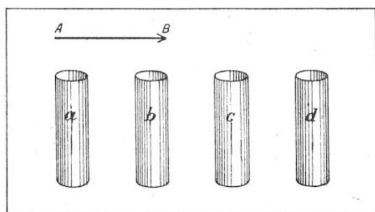
FIG. 1. — UN SYSTÈME PEUT ÊTRE A LA FOIS STABLE ET EXPLOSIF
