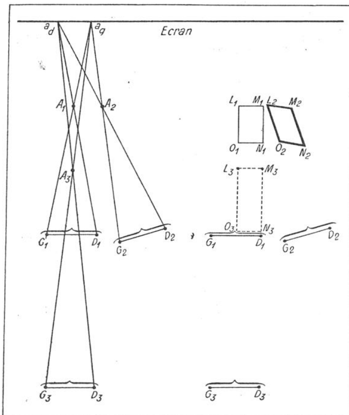
FIG. 2. — LA DÉFORMATION DU RELIEF SUIVANT LA POSITION DU SPECTATEUR
