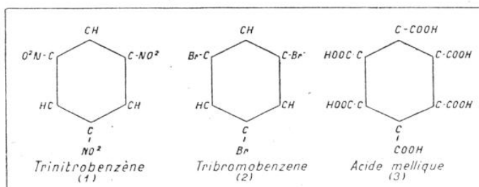
FIG. 2. — LA MOLÉCULE D'UN CORPS EXPLOSIF EST UN RÉSERVOIR D'ÉNERGIE CHIMIQUE
