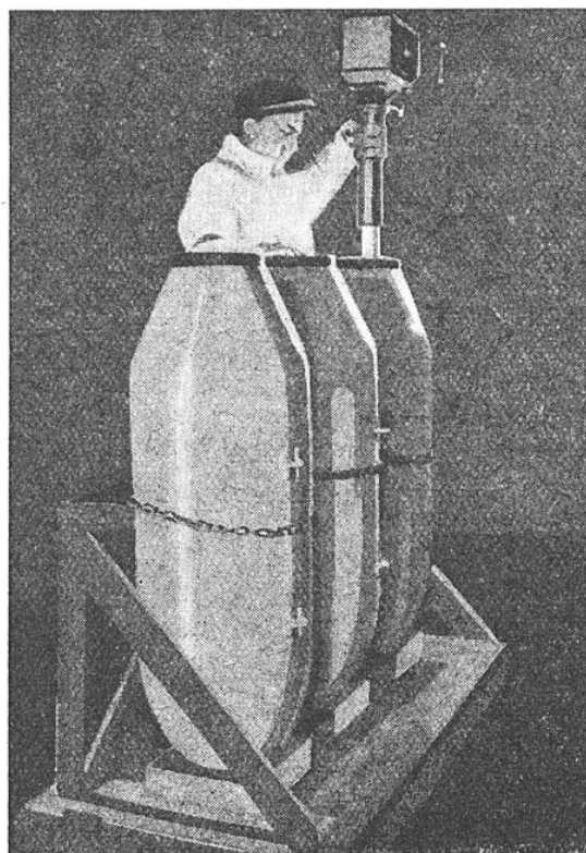
FIG. 3. — LE CHARGEMENT D'UNE BOMBE A L'AMATOL FONDU
