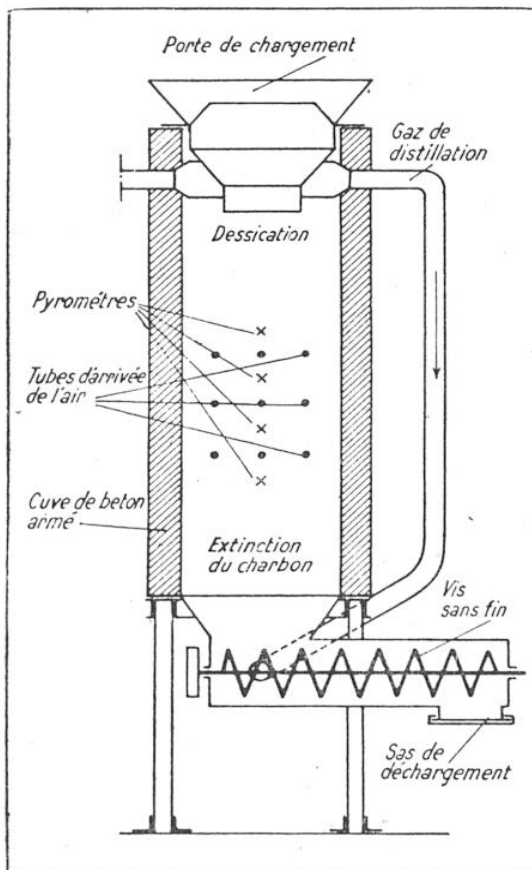
FIG. 9. — SCHÉMA DE PRINCIPE D'UNE USINE DE DISTILLATION DU BOIS DANS UN BAIN DE PLOMB EN FUSION (FOURS HARENG)
