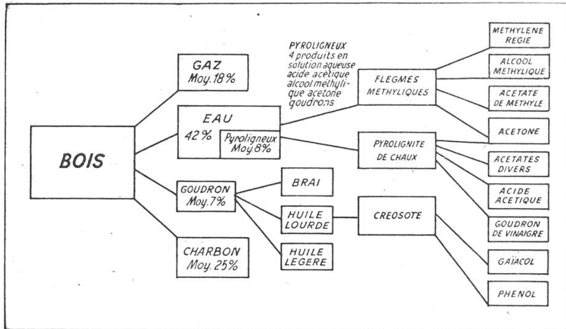
FIG. 10. — SCHÉMA MONTRANT LES PRINCIPAUX PRODUITS QUE L'ON PEUT EXTRAIRE DU BOIS PAR UNE CARBONISATION RATIONNELLE
