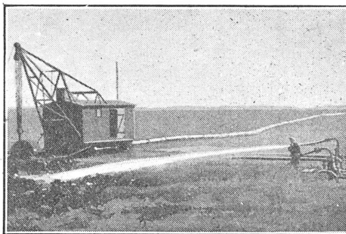
FIG. 5. — L'EXTRACTION DE LA TOURBE PAR LE PROCÉDÉ DE L'HYDROMASSE (CLASON)
