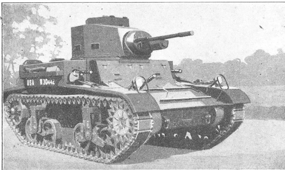
FIG. 4. — LE CHAR LÉGER M 2 A 4 DE L'INFANTERIE AMÉRICAINE
