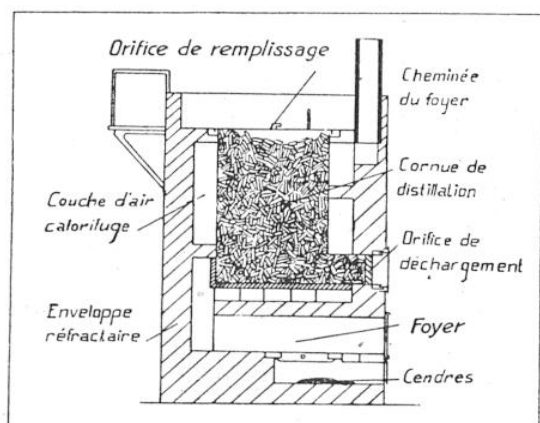
FIG. 4. — ÉLÉMENT D'UN FOUR SEMI-FIXE « CARBODISTIL » A RÉCUPÉRATION DES PRODUITS DE DISTILLATION
