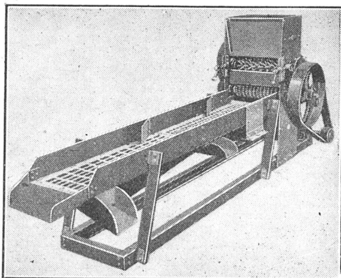
FIG. 15. CONCASSEUR MÉCANIQUE A CHARBON DE BOIS (ROLLAND) Ce concasseur comporte deux cylindres munis de couronnes de dents n'engrenant pas et tournant en sens inverse. Les brins sont triés par un tamis à secousses.
