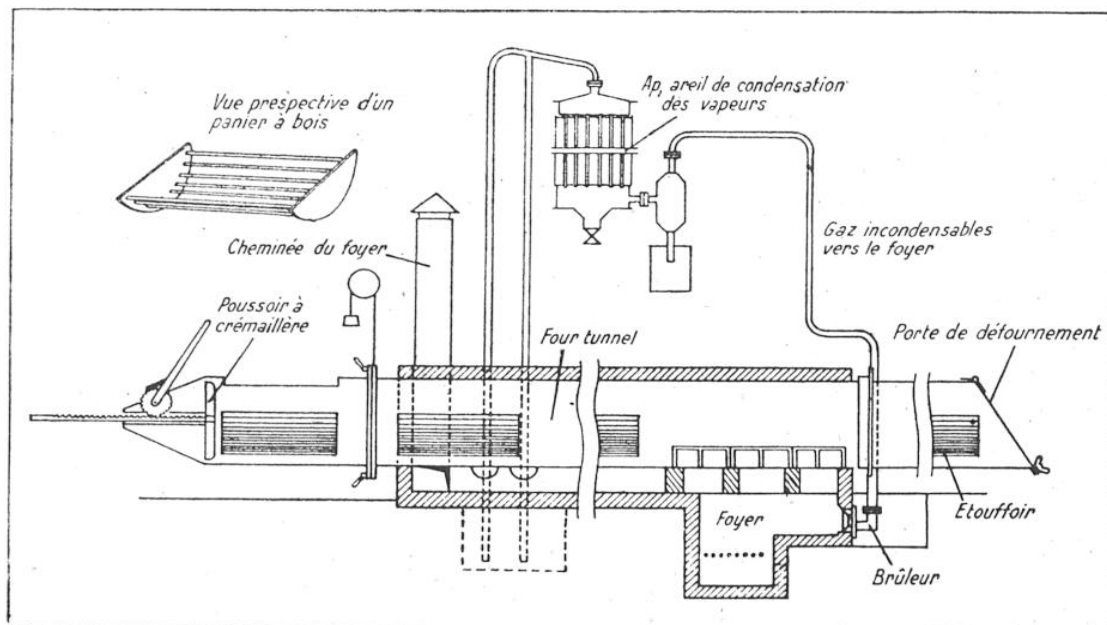
FIG. 5. — FOUR PILLARD A FONCTIONNEMENT SEMI-CONTINU ET RÉCUPÉRATION DES PRODUITS VOLATILS
