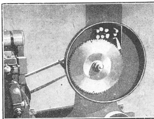
FIG. 1. — SCIE GLOPPE POUR LE DÉBITAGE DU BOIS
