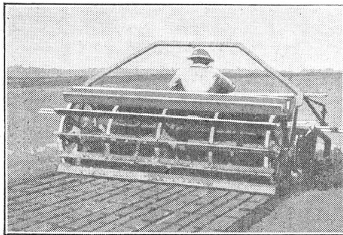
FIG. 3. — DÉCOUPAGE DE LA PULPE DE TOURBE SUR L'AIRE DE SÉCHAGE
