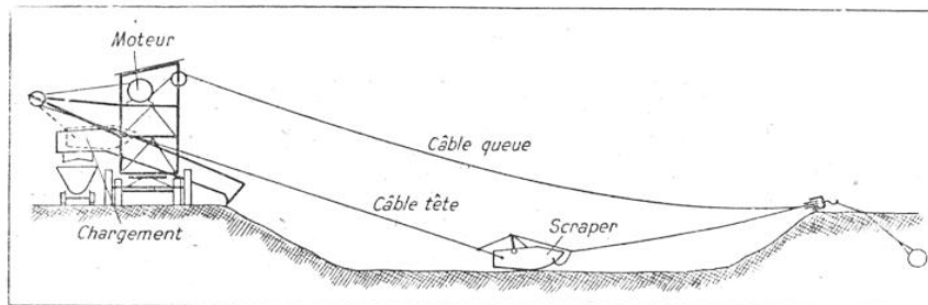
FIG. 6. — L'EXTRACTION DE LA TOURBE PAR SCRAPER
