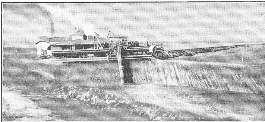
FIG. 2. — EXCAVATRICE POUR L'EXTRACTION DE LA TOURBE, EN SERVICE DANS UNE TOURBIÈRE CANADIENNE
