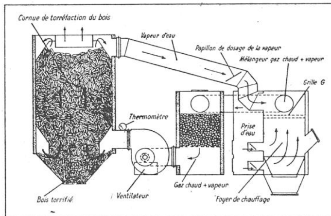
FIG. 16. — FOUR DE TORRÉFACTION DU BOIS FACEL
