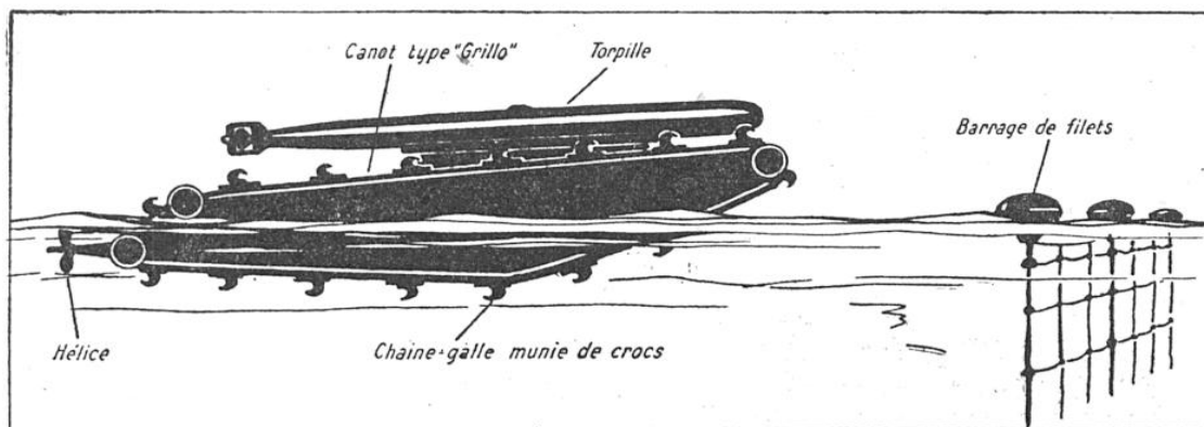
FIG. 3. — SCHÉMA D'UN TANK MARIN DU TYPE « GRILLO »
