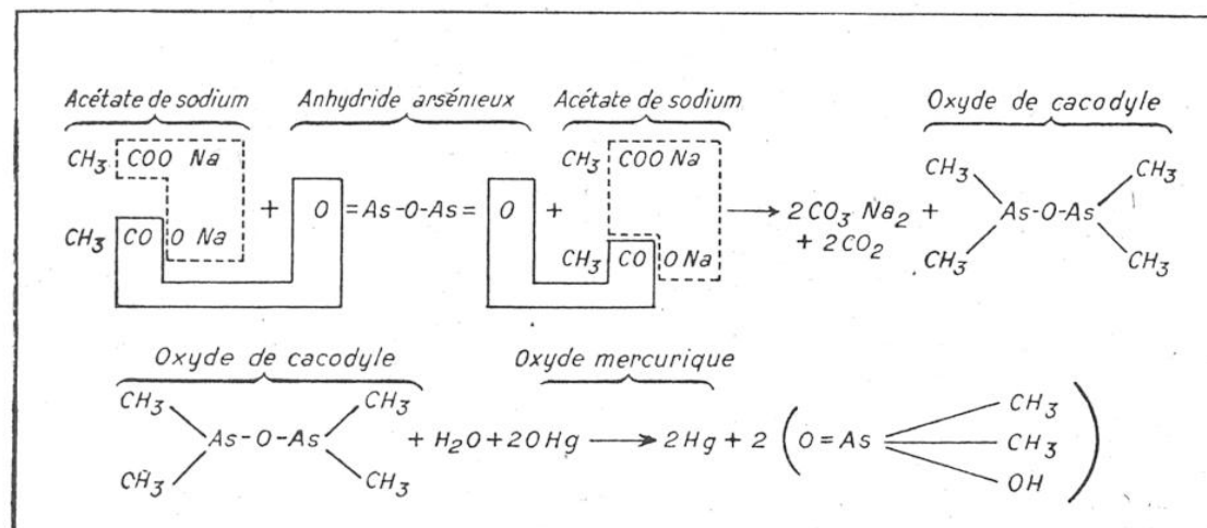
FIG. 1. — LES DEUX ÉTAPES DE LA PRÉPARATION DE L'ACIDE CACODYLIQUE
