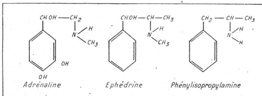
FIG. 5. — CES TROIS CORPS, ADRÉNALINE (EXTRAITE DES CAPSULES SURRÉNALES), ÉPHÉDRINE (EXTRAITE D'UNE PLANTE) ET LE PHÉNYLISOPROPYLAMINE (DE SYNTHÈSE) ONT DES PROPRIÉTÉS BIOLOGIQUES TRÈS VOISINES
