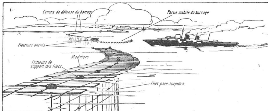
FIG. 1. — UNE ESTACADE DE DÉFENSE D'UN PORT OU D'UNE RADE
