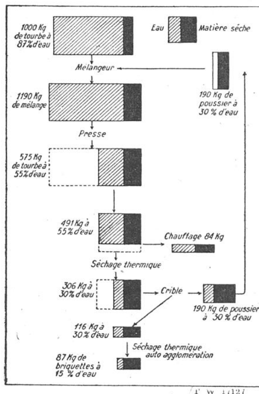
FIG. 1. — DIAGRAMME MONTRANT LA SUCCESSION DES OPÉRATIONS DANS LE PROCÉDÉ MADRUCK DE SÉCHAGE DE LA TOURBE
