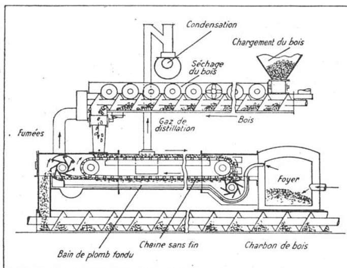
FIG. 9. — SCHÉMA DE PRINCIPE D'UNE USINE DE DISTILLATION DU BOIS DANS UN BAIN DE PLOMB EN FUSION (FOURS HARENG)
