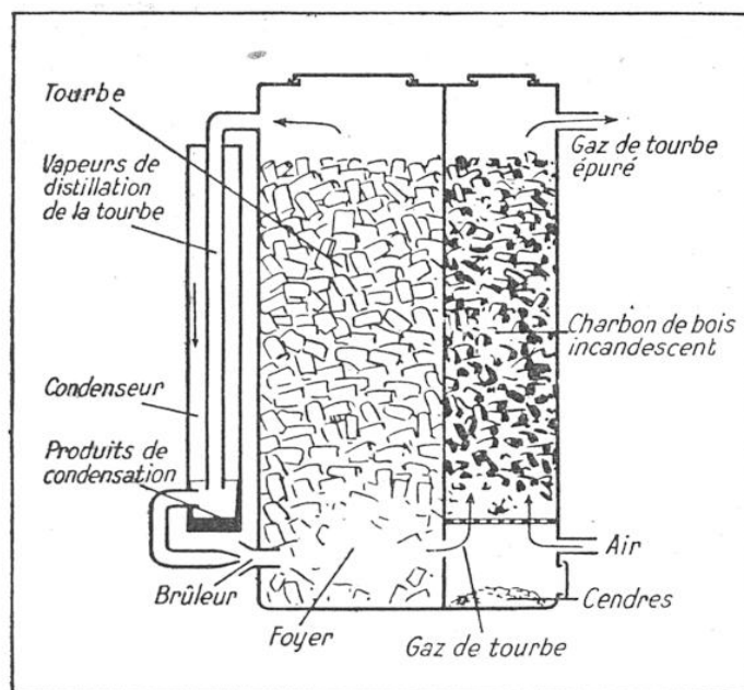
FIG. 8. — GAZOGÈNE A DEUX CUVES POUR LA GAZÉIFICATION DE LA TOURBE ET DU LIGNITE
