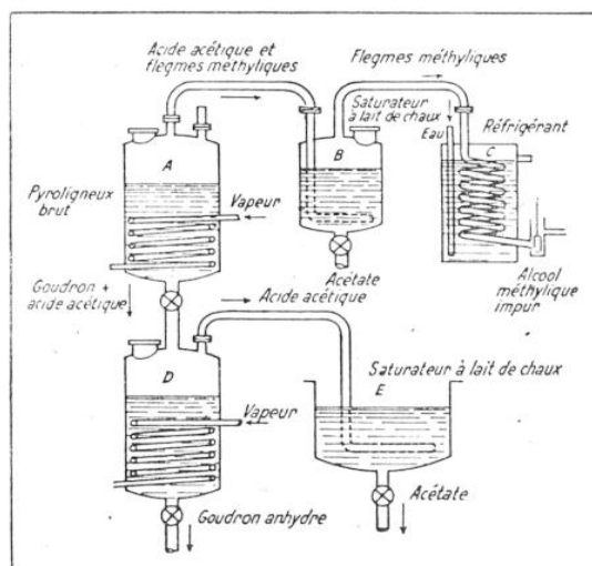
FIG. 13. — APPAREIL A TROIS CHAUDIÈRES POUR LE TRAITEMENT DU PYROLIGNEUX BRUT
