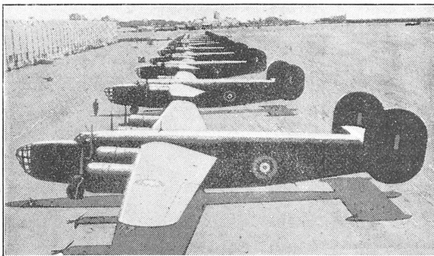
FIG. 9. — QUADRIMOTEURS DE COMBAT LOINTAIN CONSOLIDATED B-24 « LIBERATOR », ALIGNÉS DEVANT LES USINES AVANT L'EXPÉDITION EN GRANDE-BRETAGNE
