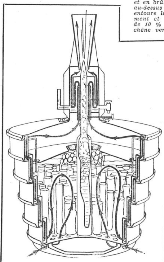
FIG. 6. — FOUR DE CARBONISATION TRANSPORTABLE A FOYER INTÉRIEUR ET RÉCUPÉRATION DES PRODUITS DE DISTILLATION (BONNECHAUX)
