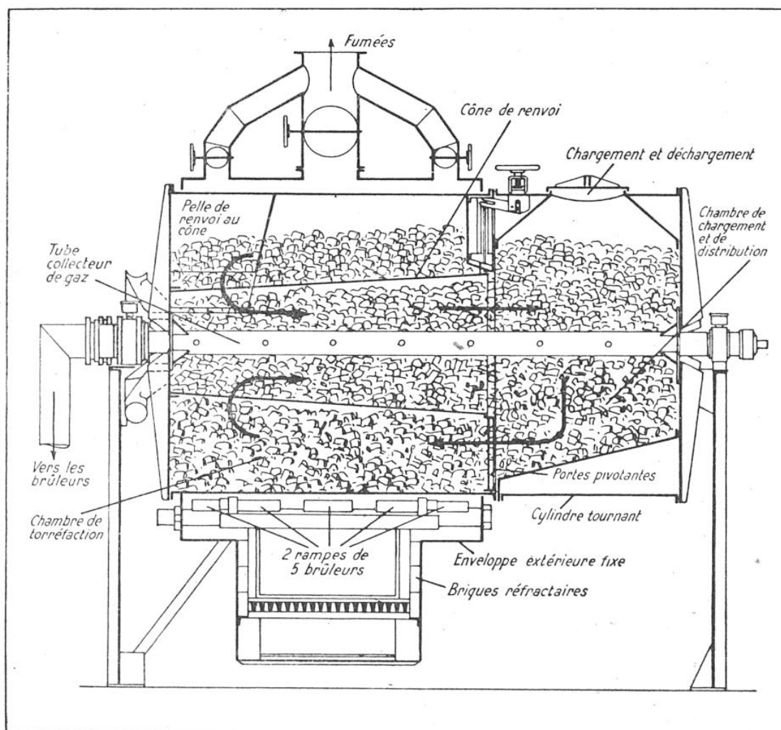
FIG. 17. — APPAREIL ROUX-DUCLOS POUR LA TORRÉFACTION DU BOIS EN VASE CLOS
