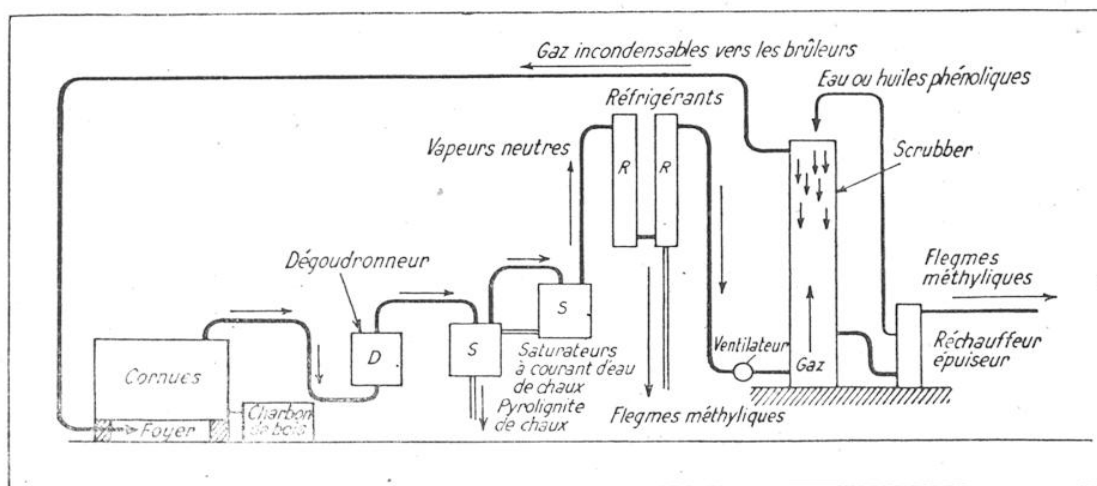
FIG. 12. — SCHÉMA D'UN CYCLE DE DISTILLATION DU BOIS AVEC FIXATION CHIMIQUE DES PRODUITS ACIDES
