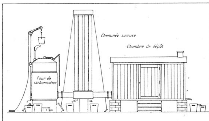
FIG. 7. — FOUR DE CARBONISATION CONTINUE A RÉCUPÉRATION COMPLÈTE FACEL
