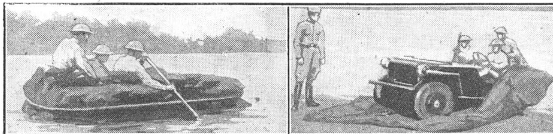
FIG. 2. — ENVELOPPÉ D'UNE BACHE, LE PYGMY FRANCHIT AISÉMENT LES COURS D'EAU
