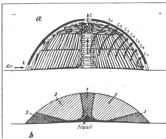
FIG. 2. — LA CARBONISATION DU BOIS DANS LES MEULES FORESTIÈRES
