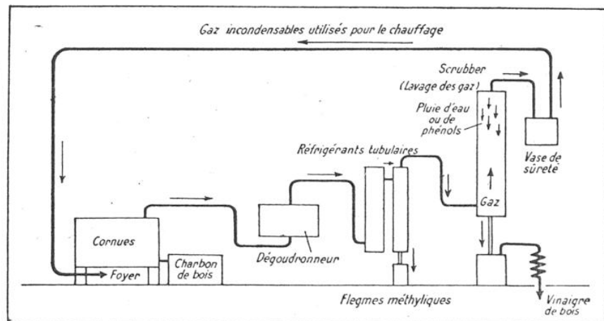
FIG. 11. — SCHÉMA D'UN CYCLE DE DISTILLATION DU BOIS AVEC CONDENSATION DIRECTE
