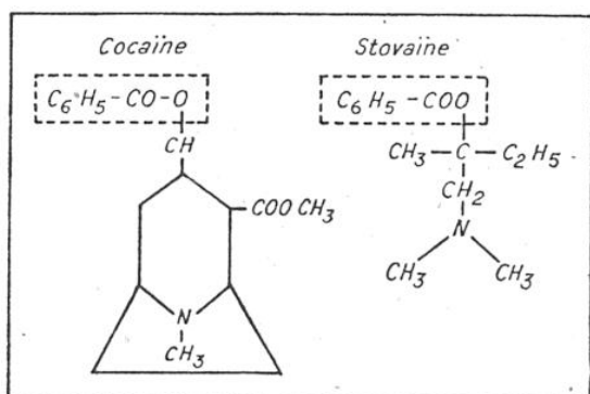
FIG. 3. — DEUX ANESTHÉSIQUES LOCAUX : LA COCAÏNE, PRODUIT NATUREL, ET LA STOVAÏNE, PRODUIT DE SYNTHÈSE
