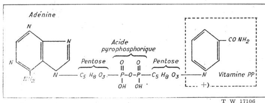
FIG. 6. — STRUCTURE DE LA COZYMASE QUI JOUE UN RÔLE CAPITAL DANS LE MÉTABOLISME DES CELLULES ANIMALES
