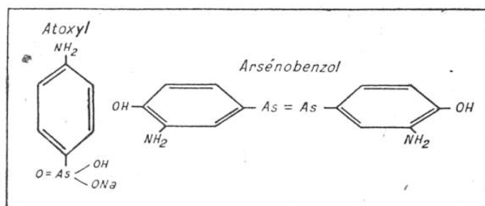
FIG. 2. — STRUCTURE DE DEUX DÉRIVÉS ORGANIQUES DE L'ARSENIC : L'ATOXYL, SPÉCIFIQUE DE LA MALADIE DU SOMMEIL, ET L'ARSÉNOBENZOL, SPÉCIFIQUE DE LA SYPHILIS
