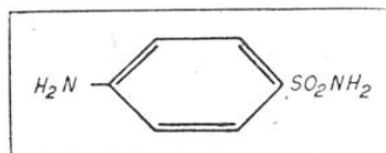
FIG. 4. — LE GROUPEMENT AMINO-BENZÈNE-SULFAMIDE AUX REMARQUABLES PROPRIÉTÉS ANTIINFECTIONNEUSES
