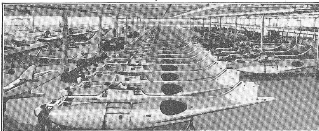
FIG. 8. — LA FABRICATION EN SÉRIE DES HYDRAVIONS BIMOTEURS CONSOLIDATED P B Y « CATALINA » : Cet appareil à grand rayon d'action est utilisé non seulement par la Marine américaine, mais par les escadrilles du Commandement aérien des côtes en Grande-Bretagne. Il sert en particulier au convoyage aérien des navires.
