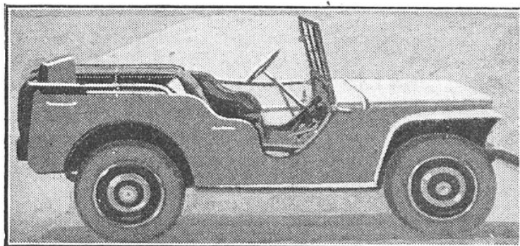
FIG. 1. — LA VOITURE « TOUTS TERRAINS » PYGMY
