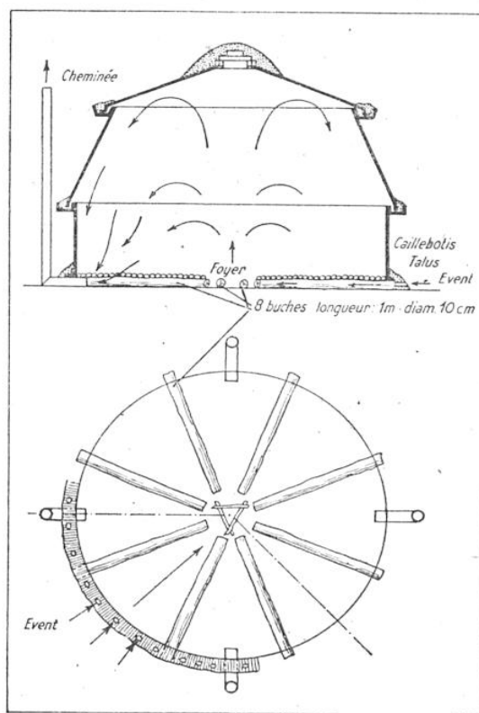
FIG. 3. — FOUR A CARBONISER DÉMONTABLE DES EAUX ET FORÊTS
