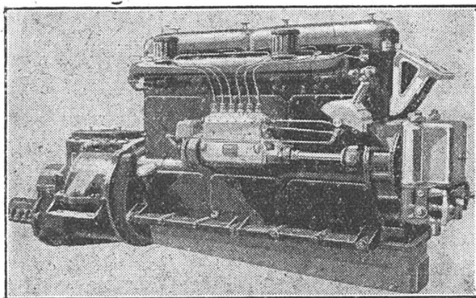
FIG. 6. — GROUPE DE PROPULSION DIESEL MARIN 6 CYLINDRES DE 85 CHEVAUX
