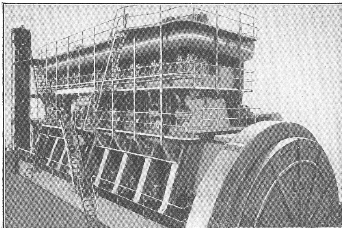
FIG. 1. — L'UN DES MOTEURS DIESEL DE 24 000 CH DE LA CENTRALE DE COPENHAGUE (BURMEISTER ET WAIN'S) T W 16457
