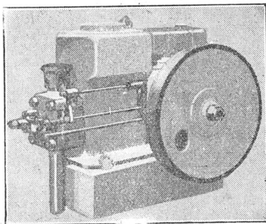
FIG. 2. — PETIT MOTEUR DIESEL HORIZONTAL A QUATRE TEMPS, DE 4 CHEVAUX
