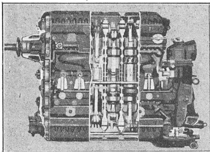
FIG. 9. — COUPE DU MOTEUR DIESEL D'AVIATION JUNKERS « JUMO 205 »
