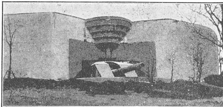
FIG. 3. — CANON LOURD ALLEMAND SOUS CASEMATE DESTINÉ A LA DÉFENSE DE LA CÔTE BELGE
