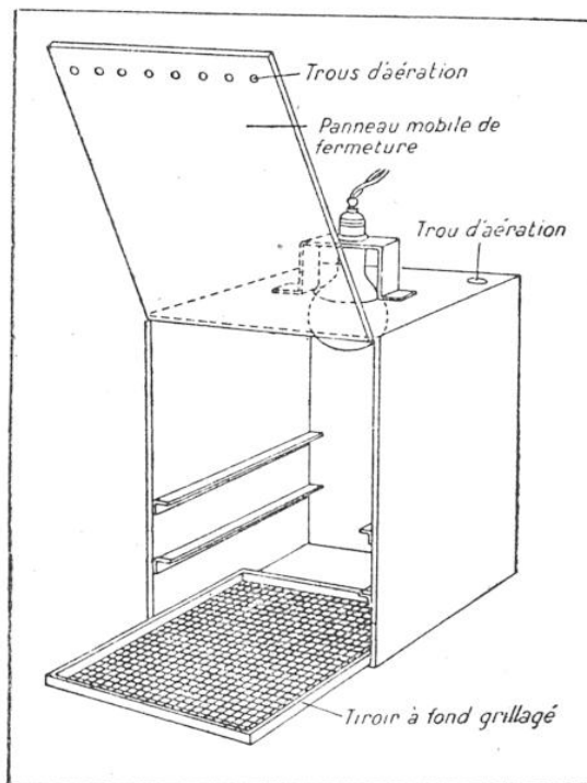
FIG. 2. — UNE PETITE ÉTUVE DE SÉCHAGE PAR RAYONS INFRAROUGES
