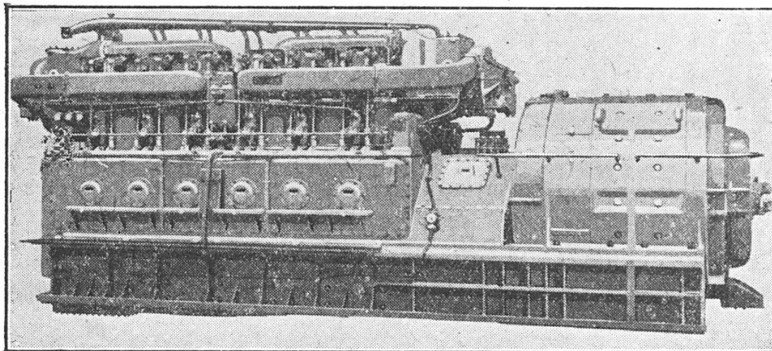
FIG. 5. — MOTEUR DIESEL 12 CYLINDRES A QUATRE TEMPS DE 2 200 CH DE LA LOCOMOTIVE DIESEL-ÉLECTRIQUE DES CHEMINS DE FER ROUMAINS T W 16452
