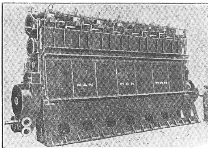
FIG. 7. — MOTEUR DIESEL DE 2 600 CH DU CARGO ALLEMAND « WUPPERTAL »
