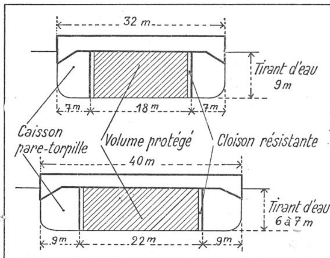
FIG. 2. — COMPARAISON DU NAVIRE DE 32 MÈTRES ET DU NAVIRE DE 40 MÈTRES DE LARGEUR DU POINT DE VUE DE LA PROTECTION CONTRE LA TORPILLE SOUS-MARINE
