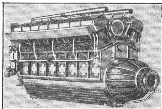
FIG. 8. — MOTEUR DIESEL A 16 CYLINDRES DE 900-1 200 CH DU ZEPPELIN « HINDENBURG » (MERCEDES-BENZ)
