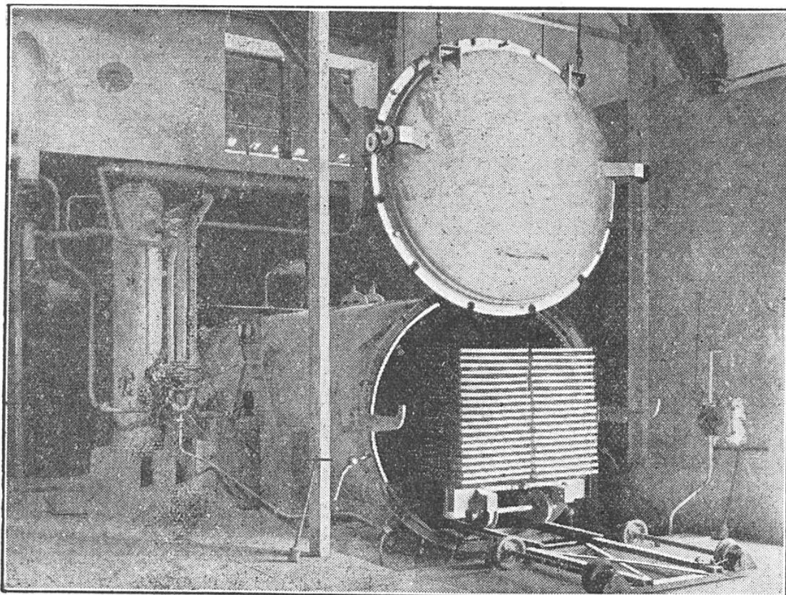
FIG. 5. — UN CUISEUR-BLANCHISSEUR POUR LE TRAITEMENT DES LÉGUMES DANS UNE USINE DE FABRICATION DE LÉGUMES DÉSHYDRATÉS (ET. BARBIER ET DAUPHIN)
