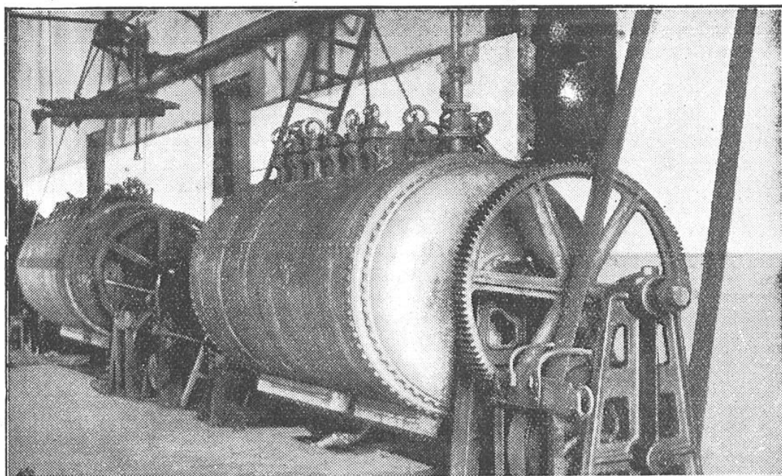
FIG. 2. — UNE BATTERIE D'AUTOCLAVES A PANIER DE 1.500 KG DE CAPACITÉ
