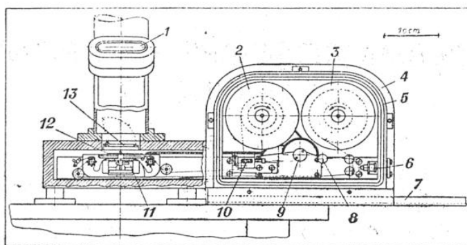
FIG. 2. — SCHÉMA D'ENSEMBLE DE LA CAMERA ADAPTÉE A L'HYPER-MICROSCOPE ÉLECTRONIQUE
