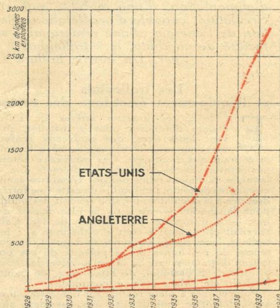
FIG. 2. — LONGUEURS DE LIGNES DE TROLLEYBUS EXPLOITÉES DANS DIVERS PAYS
