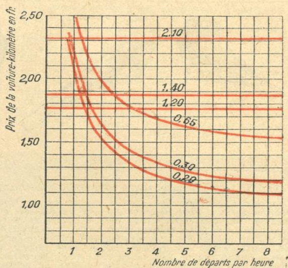
FIG. 4. — DÉPENSES COMPARÉES DU TROLLEYBUS ET DE L'AUTOBUS PAR KILOMÈTRE PARCOURU EN FONCTION DE L'INTENSITÉ DU TRAFIC
