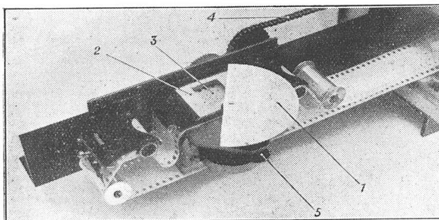
FIG. 5. — LE DISPOSITIF DE GUIDAGE DU FILM POUR LA CAMERA DE L'HYPERMICROSCOPE ÉLECTRONIQUE
