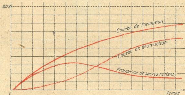
FIG. 2. — LA FORMATION ET LA DESTRUCTION DES SUCRES DANS L'HYDROLYSE À CHAUD DE LA CELLULOSE (CHARLES MEUNIER)
