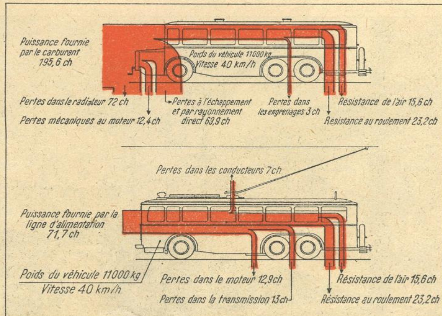
FIG. 9. — LE BILAN DES PERTES D'ÉNERGIE DANS UN AUTOBUS A ESSENCE ET DANS UN TROLLEYBUS
