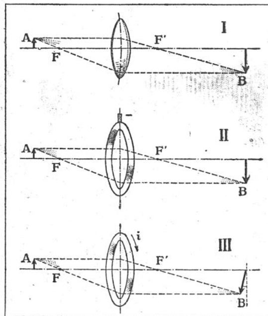
FIG. 1. — SCHÉMA DE PRINCIPE DE DIFFÉRENTES LENTILLES
