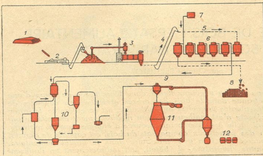
FIG. 1. — LA FABRICATION DU SUCRE DE BOIS PAR LE PROCÉDÉ BERGIUS
