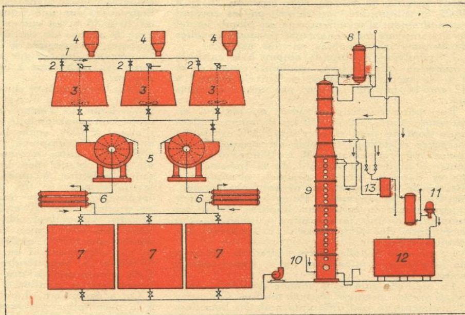
FIG. 7. — SCHÉMA DU DISPOSITIF SCHOLLER POUR LA FERMENTATION ÉTHYLIQUE DU MOUT SUCRÉ OBTENU PAR HYDROLYSE
