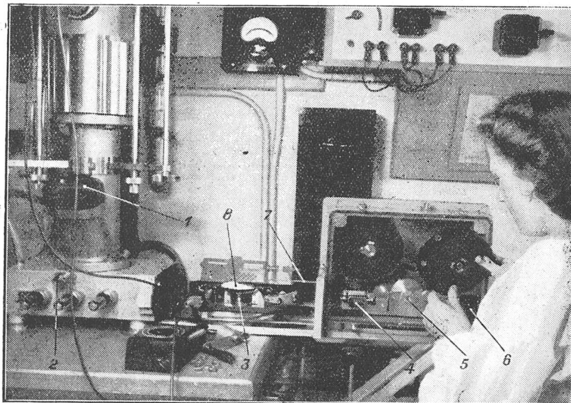
FIG. 3. — VUE INTÉRIEURE DE LA CAMERA, A LA BASE DE L'HYPERMICROSCOPE ÉLECTRONIQUE
