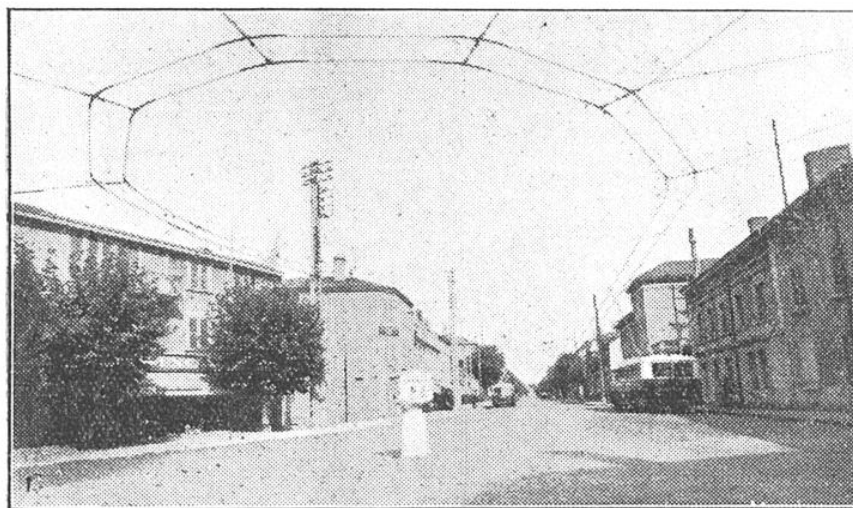
FIG. 6. — BOUCLE DE RETOURNEMENT D'UNE LIGNE DE TROLLEYBUS A LYON (VÉTRA)
