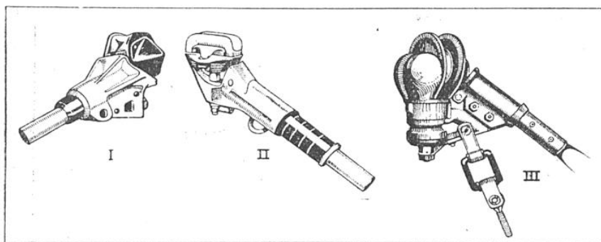
FIG. 5. — TROIS DISPOSITIFS DE PRISE DE COURANT SUR LA VOIE AÉRIENNE
