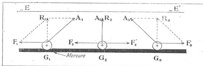
FIG. 5. — L'ÉQUILIBRE DES FORCES D'ATTRACTION ET DE RÉPULSION DANS UNE COLLECTION DE GRAINES FLOTTANTES SOUMISES A UN CHAMP ÉLECTRIQUE VERTICAL
