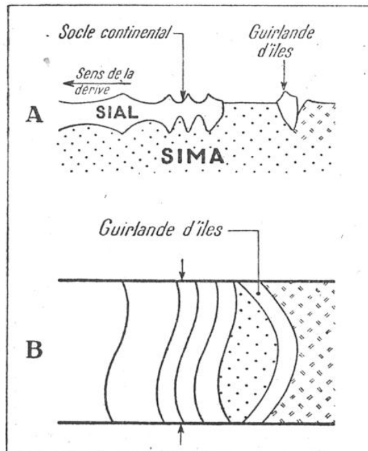
FIG. 9. — SCHÉMA DE LA GENÈSE DES GUIRLANDES D'ÎLES, SUIVANT LA THÉORIE DE WEGENER
