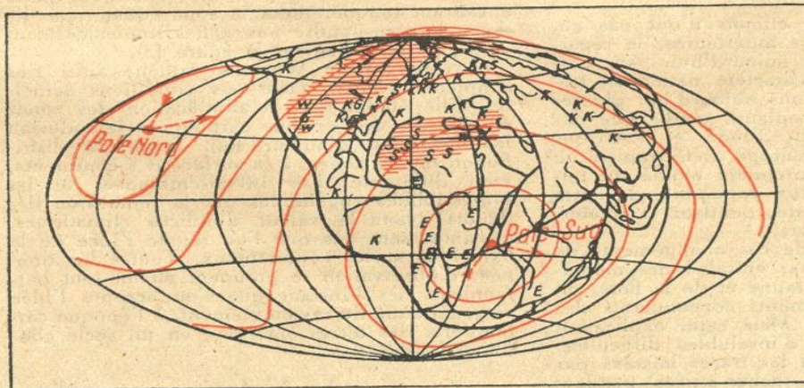
FIG. 13. — LA RÉPARTITION DES TEMPÉRATURES AU CARBONIFÈRE, RÉVÉLÉE PAR LES DÉPÔTS QUI DATENT DE CETTE PÉRIODE
