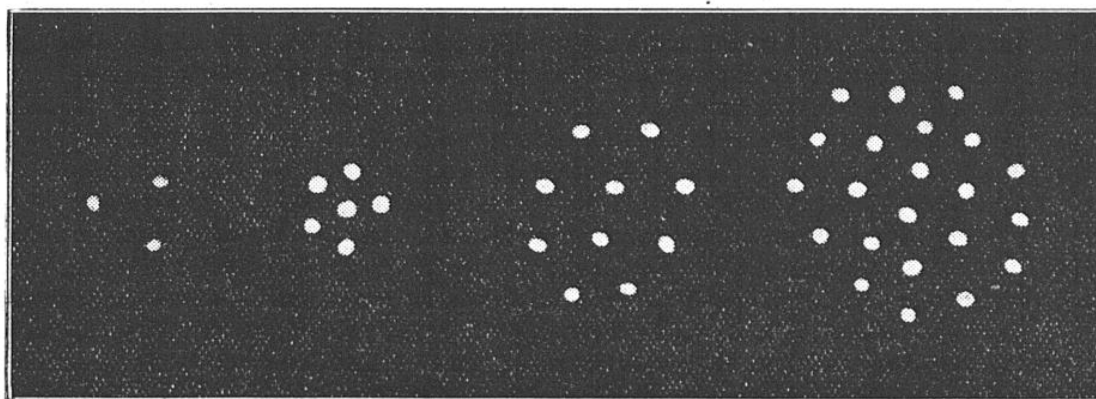
FIG. 4. — RÉPARTITION SPONTANÉE DE GRAINES FLOTTANT SUR LE MERCURE ET SOUMISES A UN CHAMP ÉLECTRIQUE VERTICAL
