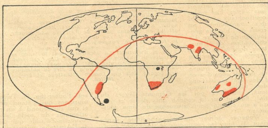
FIG. 12. — LES TRACES DE GLACIATION SUR LES CONTINENTS ACTUELS A L'ÉPOQUE PERMO-CARBONIFÈRE, D'APRÈS WEGENER
