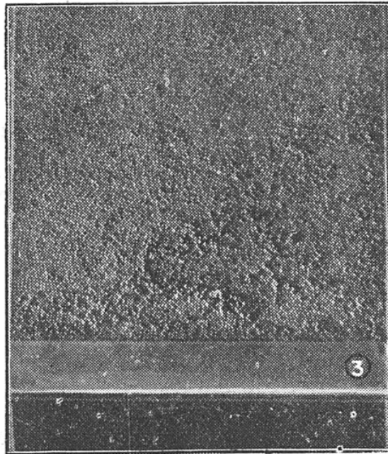
FIG. 2. — GRAINES RONDÉS DE COLZA ÉTENDUES EN LAME UNIPARTICULAIRE A LA SURFACE DU MERCURE En 1, la nappe est « distendue »; elle présente des trous, la quantité de graines étant insuffisante pour couvrir la totalité de la surface. En 2, la surface est critique : comprimée latéralement par la bande de papier mobile visible dans le bas de la figure, les graines commencent à grimper les unes sur les autres. En 3, le point critique est dépassé; de nombreuses graines s'échappent en hauteur.
