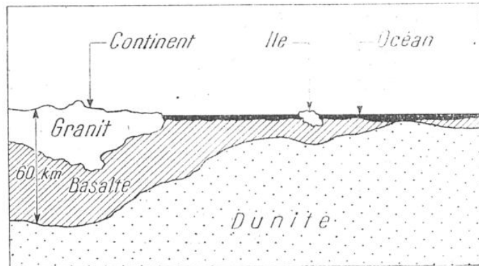
FIG. 6. — COUPE DE L'ÉCORCE TERRESTRE À TRAVERS UN SOCLE CONTINENTAL (À GAUCHE) ET UN FOND OcéANIQUE (À DROITE), D'APRÈS WEGENER
