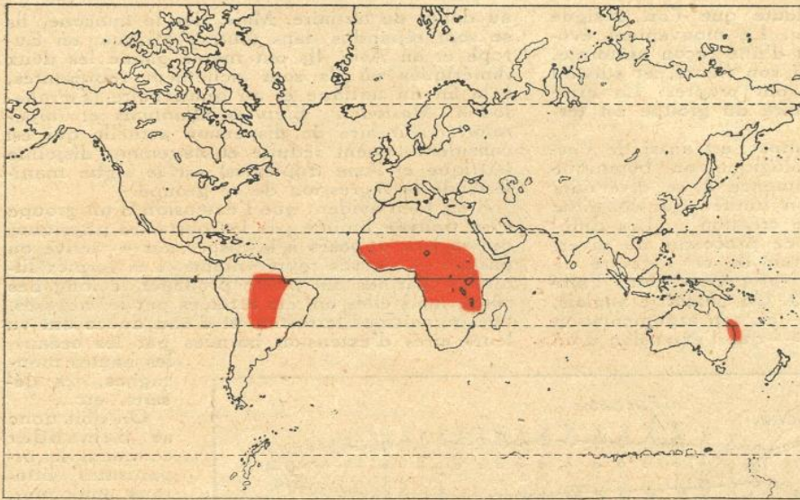
FIG. 2. — LA RÉPARTITION DES DIPNEUSTES ACTUELS A LA SURFACE DU GLOBE
