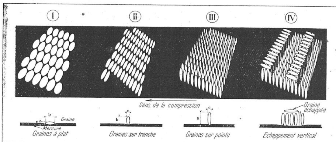
FIG. 3. — IL EXISTE TROIS POINTS CRITIQUES AVEC LES NAPPES UNIPARTICULAIRES FORMÉES DE GRAINES A TROIS AXES INÉGAUX
