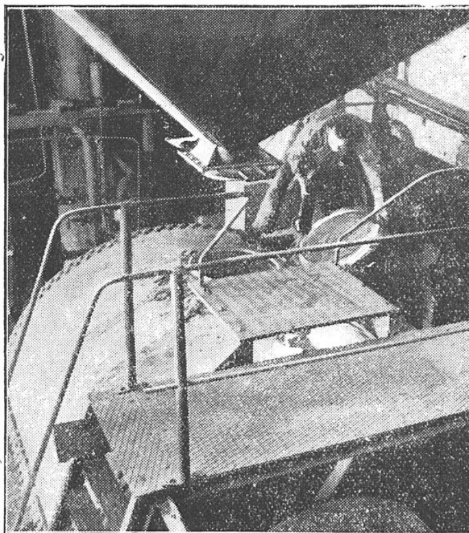
FIG. 3. — CUVE POUR L'HYDROLYSE DU BOIS PAR LE PROCÉDÉ MEUNIER
