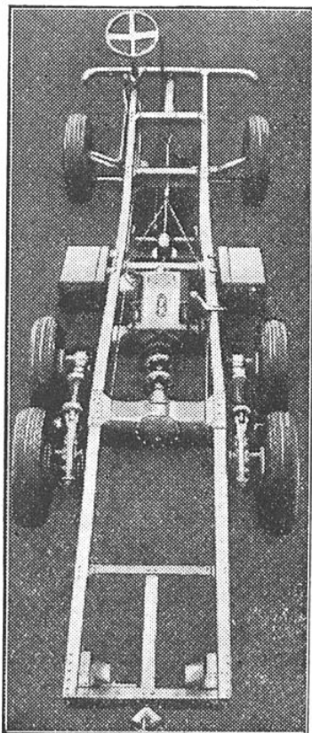
FIG. 8. — LE CHASSIS D'UN TROLLEYBUS ÉQUIPÉ DE SON MOTEUR ÉLECTRIQUE (RHEINISCH-WESTFÄLISCHES ELEKTRIZITÄTSWERK)
