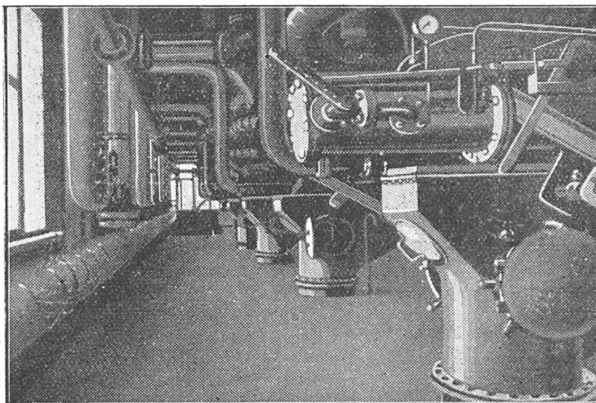
FIG. 5. — LA PARTIE INFÉRIEURE DES CUVES DE TRAITEMENT DU BOIS (PROCÉDÉ SCHOLLER)
