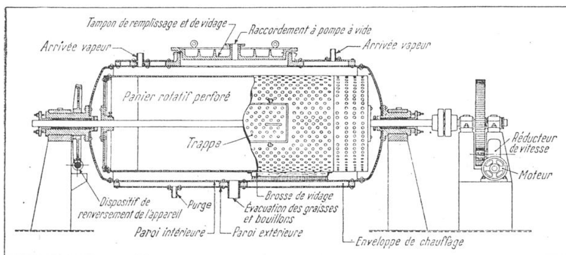
FIG. 1. — SCHÉMA D'UN CUISEUR-DESSICCATEUR À PANIER ROTATIF POUR LE TRAITEMENT DES DÉCHETS ANIMAUX (SYSTÈME MARLION)
