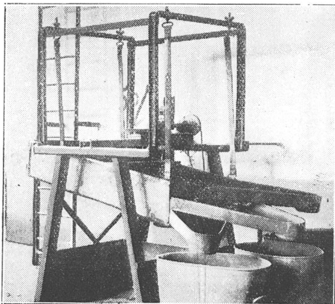
FIG. 4. — APPAREIL DE CLASSEMENT DES PRODUITS DE BROYAGE DES COQUILLES D'HUITRES ET DE MOULES
