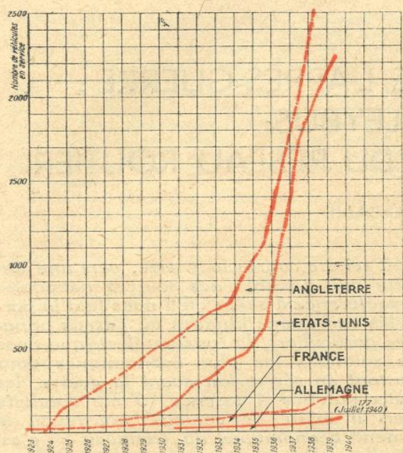
FIG. 1. — COURBES MONTRANT LE DÉVELOPPEMENT DE LA CONSTRUCTION DES TROLLEYBUS DANS DIVERS PAYS (NOMBRE DE VÉHICULES EN SERVICE)
