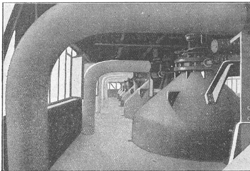
FIG. 4. — UNE BATTERIE DE PERCOLATEURS DANS UNE USINE ALLEMANDE D'HYDROLYSE DE BOIS SELON LE PROCÉDÉ SCHOLLER
