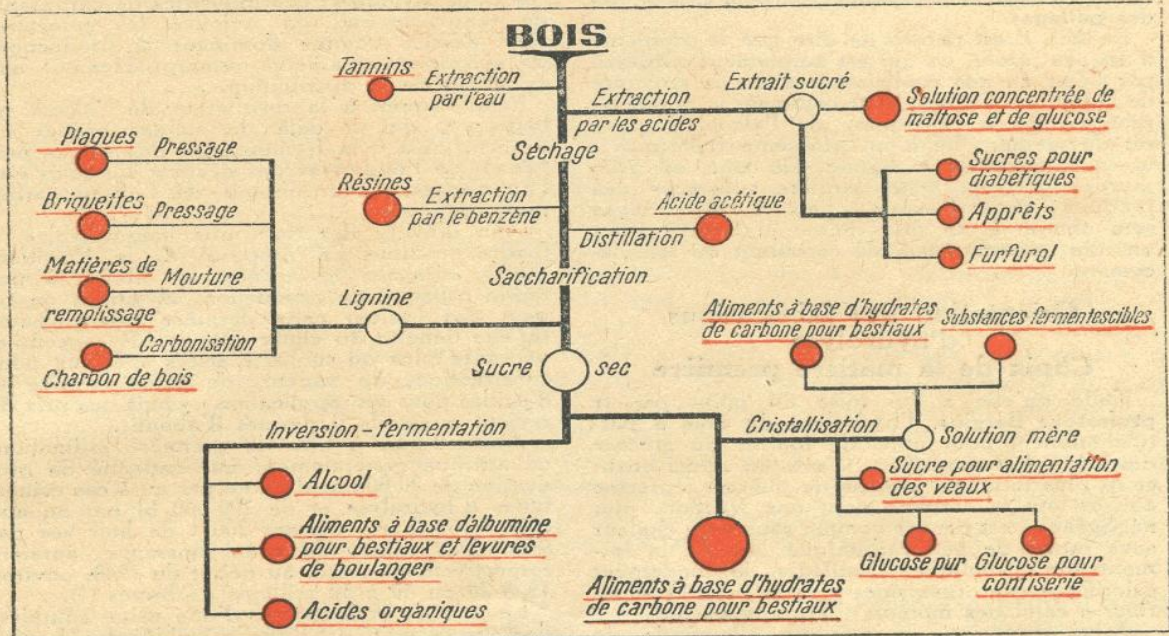
FIG. 8. — ENSEMBLE DES PRODUITS POUVANT ÊTRE OBTENUS PAR LE PROCÉDÉ BERGIUS D'HYDROLYSE DE LA CELLULOSE
