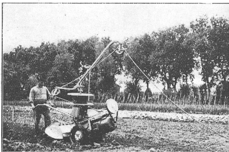
FIG. 1. — VUE D'ENSEMBLE DU MOTOCULTEUR ÉLECTRIFIÉ
