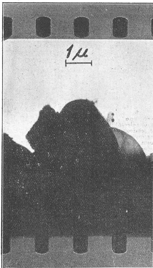
FIG. 6. — UNE PHASE DE LA FORMATION DE GROS CRISTAUX D'OR, A PARTIR DE MICROCRISTAUX, PAR CHAUFFAGE A 1 000° C
