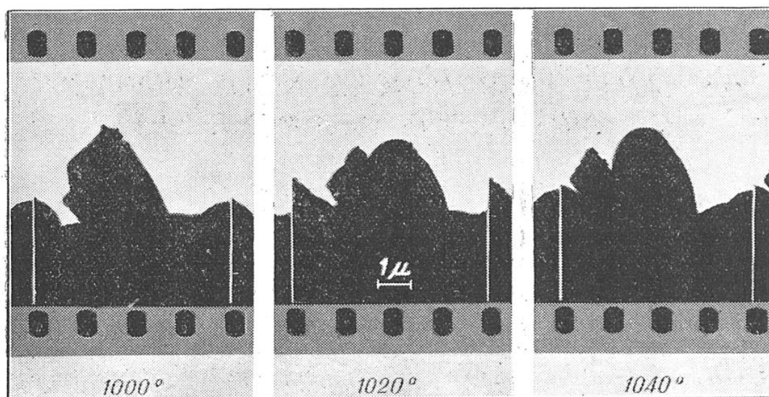
FIG. 7. — IMAGES FORTEMENT GROSSIES, EXTRAITES DU PREMIER FILM RÉALISÉ A L'AIDE DE L'HYPERMICROSCOPE ELECTRONIQUE
