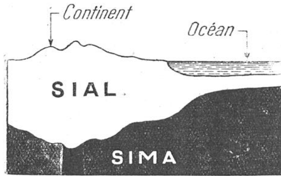
FIG. 5. — SCHÉMA DE L'« ISOSTASIE », D'APRÈS AIRY
