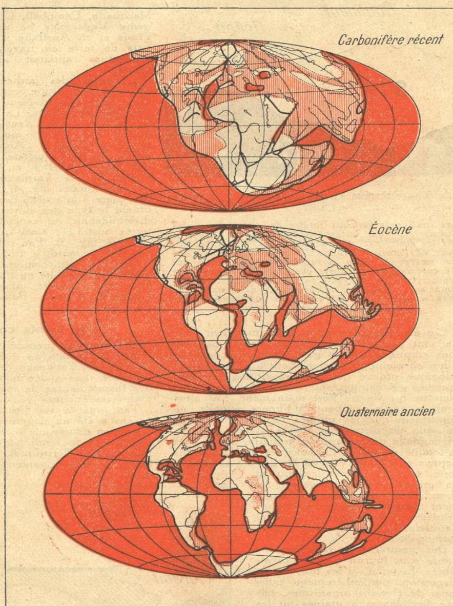
FIG. 7. — RECONSTITUTION DU GLOBE A TROIS ÉPOQUES
