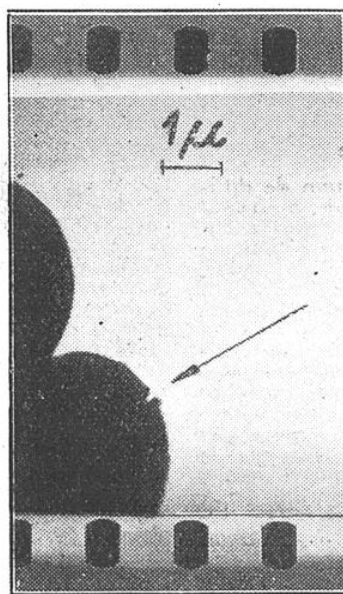
FIG. 8. — IMAGE EXTRAITE D'UN FILM SUR LA FUSION DE FINES PARTICULES D'URANIUM
