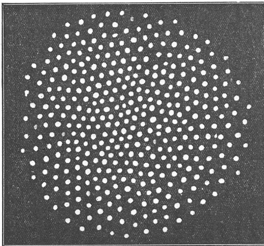
FIG. 6. — UNE GRANDE NAPPE UNIPARTICULAIRE, MONTRANT LA RÉPARTITION REMARQUABLE DES GRAINES FLOTTANTES SOUS L'ACTION D'UN CHAMP VERTICAL.
