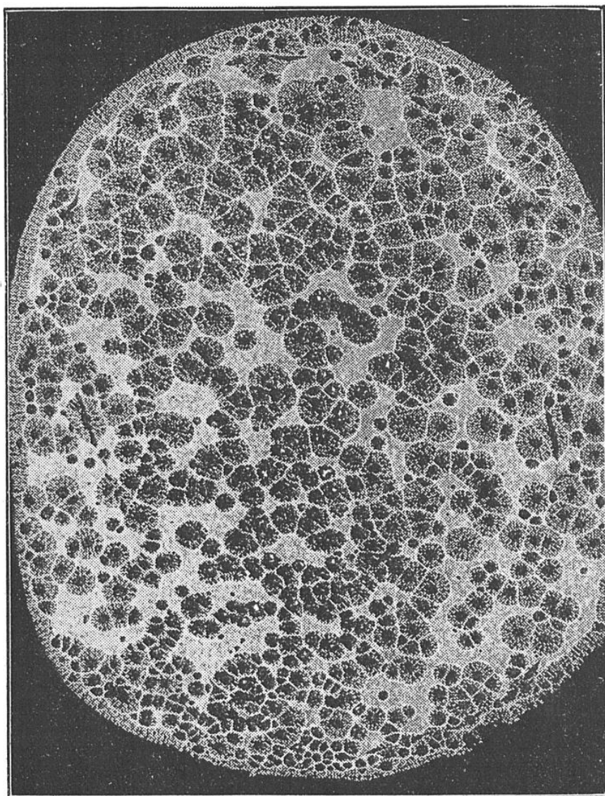
FIG. 1. — LAME MOLÉCULAIRE D'HUILE DE LIN A LA SURFACE DE L'EAU Les parties claires mesurent 1/100\,000 de mm d'épaisseur et sont formées de cinq couches de molécules; les parties sombres représentent la zone unimoléculaire. Elles sont entourées de fines gouttelettes en chapelet.
