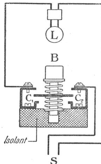
FIG. 7. — SCHÉMA DE MONTAGE DU BOUTON-CONCIERGE
