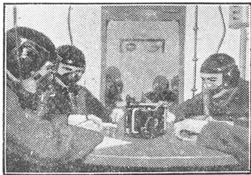
FIG. 6. — L'INTÉRIEUR D'UNE CHAMBRE DE DÉPRESSION MOBILE POUR LA MESURE DES « RÉSERVES DE TEMPS » DES PILOTES
