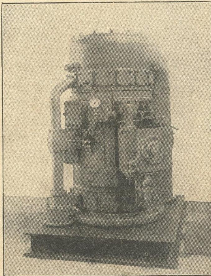
FIG. 12.— GÉNÉRATEUR PESCARA DE 450 CHEVAUX, POUR LOCOMOTIVE T W 40029
