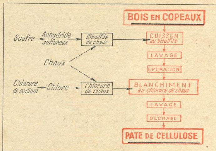
FIG. 4. — SCHÉMA DE LA FABRICATION DE LA PÂTE DE CELLULOSE
