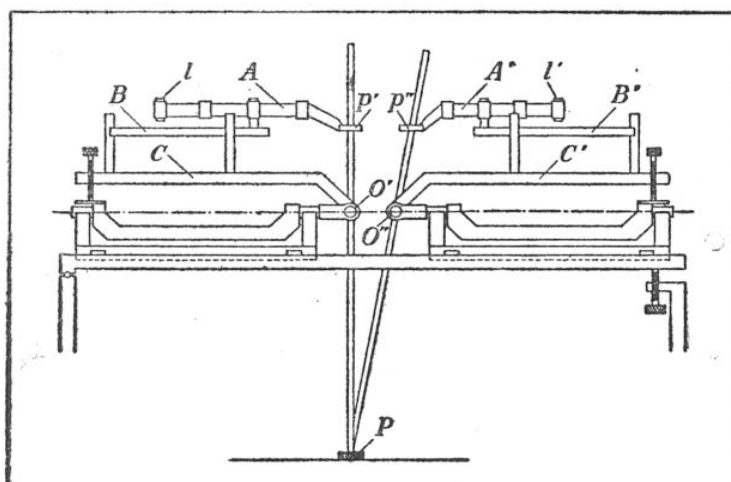
FIG. 2. — COUPE SIMPLIFIÉE DE L'AUTOGRAPHE WILD A 6
