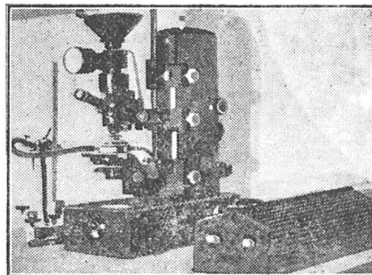
FIG. 5. — CHAMBRE DE DÉPRESSION MICROSCOPIQUE POUR L'ÉTUDE DU COMPORTEMENT DES CELLULES VIVANTES SOUS PRESSION RÉDUITE
