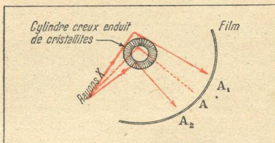
FIG. 13. — PRINCIPE DE LA MESURE DE LA DIMENSION DES CRISTALLITES (MÉTHODE DE BRILL)
