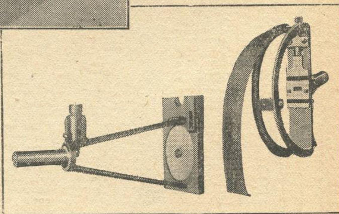
T W 40031 FIG. 10. — DEUX MODÈLES DE PORTE-FILMS POUR L'ÉTUDE CRISTALLOGRAPHIQUE PAR LA DIFFRACTION DES RAYONS X
