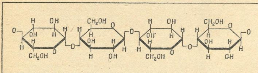
FIG. 3. — FRAGMENT D'UNE CHAÎNE CELLULOSIQUE
