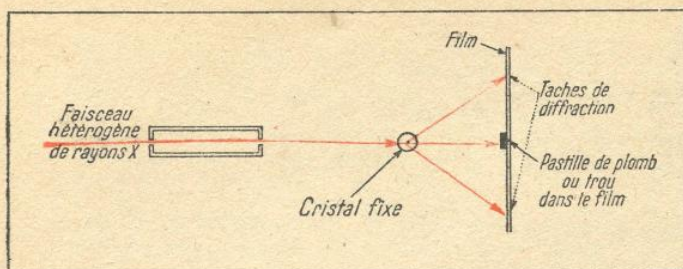
FIG. 2. — PRINCIPE DE LA MÉTHODE DE LAUE
