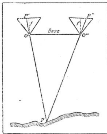
FIG. 1. — PRINCIPE DE LA PHOTOGRAPHIE STÉRÉOSCOPIQUE
