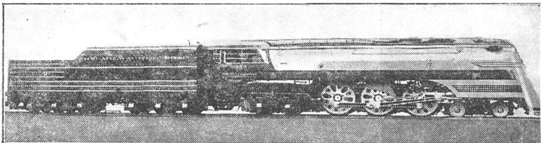
FIG. 5. — LOCOMOTIVE A VAPEUR AMÉRICAINE TYPE 232 POUR TRAINS RAPIDES, CONSTRUITE EN 1928 T W 40023 Charge des essieux moteurs : 33 tonnes. Surface de grille : 9 m 2 . Poids de la locomotive seule : 187,5 t. Poids du tender chargé : 167 t (75 m 3 d'eau et 22,5 t de charbon).
