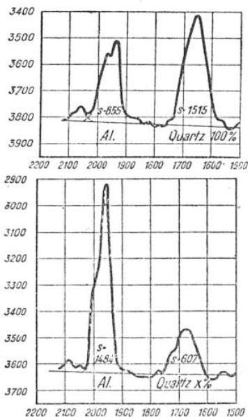
FIG. 11. - COURBES PHOTOMÉTRIQUES DES RAIES SERVANT AU DOSAGE DU QUARTZ
