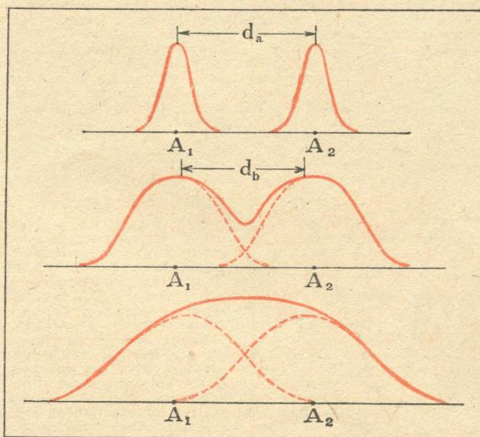
FIG. 14. — LE DÉDOUBLEMENT DES RAIES POUR L'ÉVALUATION DE LA DIMENSION DES CRISTALLITES
