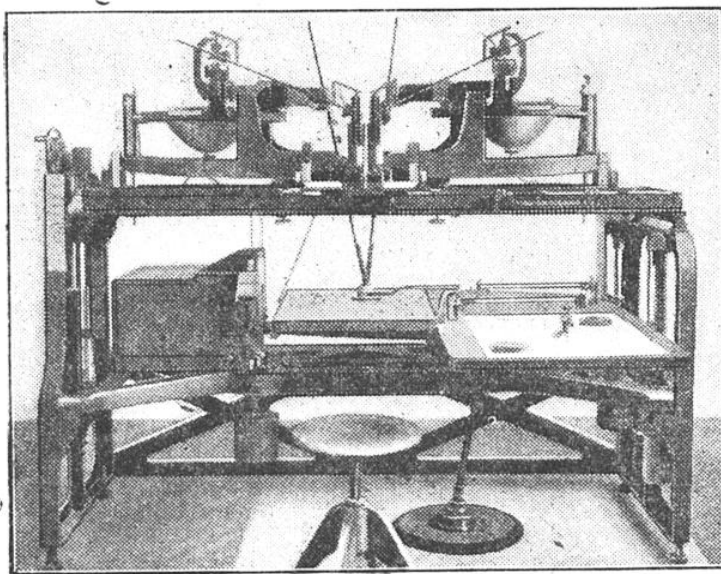
FIG. 3. — L'AUTOGRAPHE WILD A 6
