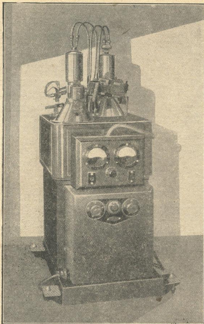
T W 40030 FIG. 9. — ENSEMBLE D'UN GROUPE POUR LA RADIOCRISTALLOGRAPHIE IN- DUSTRIELLE
