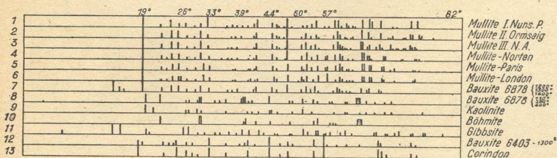
FIG. 8. — INTENSITÉS RELATIVES DES RAIES DE SPECTRES DE POUDRES
