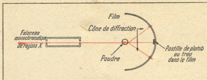
FIG. 6. — PRINCIPE DE LA MÉTHODE DE DEBYE-SCHERRER OU MÉTHODE DES POUDRES
