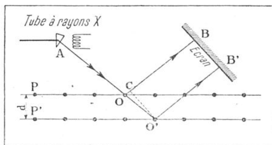
FIG. 1. — SCHÉMA DE PRINCIPE DE LA DIFFRACTION DES RAYONS X
