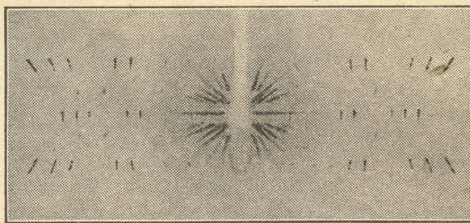
FIG. 4 et 5. — PRINCIPE DE LA MÉTHODE DE BRAGG OU DU CRISTAL TOURNANT ET DIAGRAMME DU SEL GEMME
