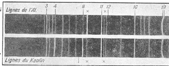
FIG. 12. — SPECTRES DESTINÉS AU DOSAGE DU QUARTZ
