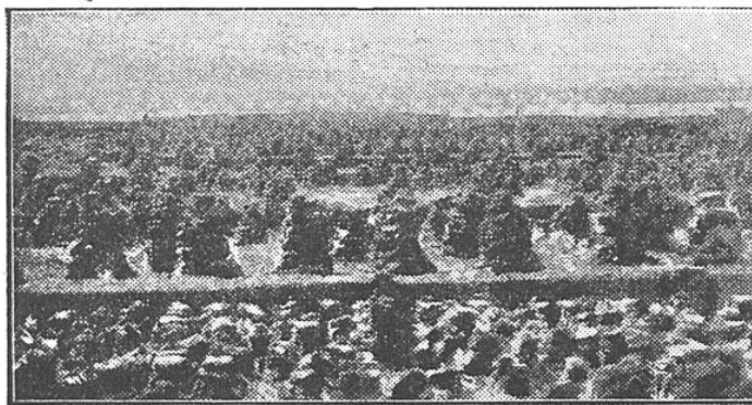
FIG. 6. — ASPECT D'UNE TOURBIÈRE SUÉDOISE AU COURS DE L'ÉTÉ Les mottes de tourbe sont montées en cheminées pour assurer une dessiccation rapide.
