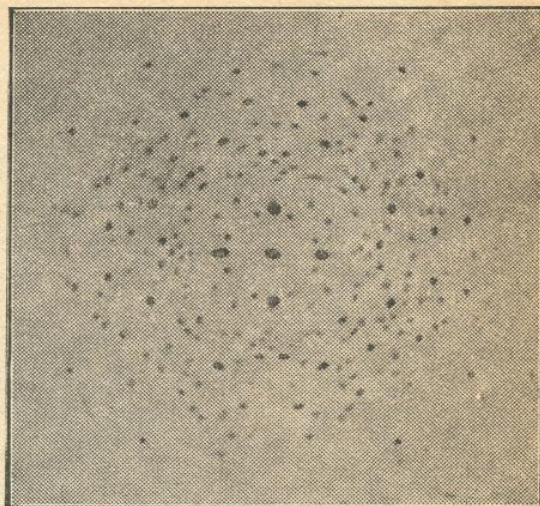
FIG. 3. — UN DIAGRAMME DE LAUE (BOLÉITE QUADRATIQUE, D'APRÈS M. R. HOCART)
