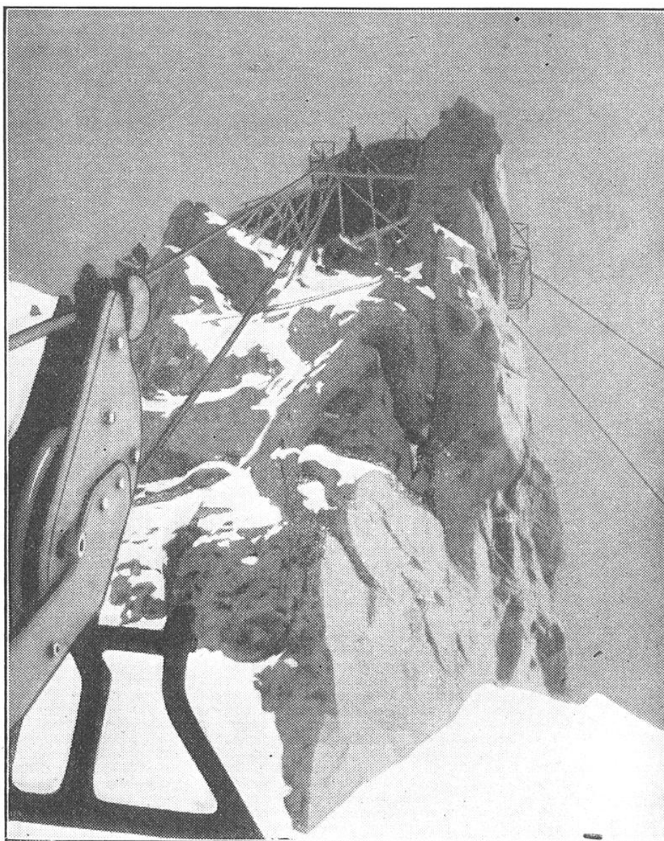
FIG. 4. — LE « GENDARME » D'ARRIVÉE ET SES PASSERELLES AU COL DU MIDI, STATION TERMINALE DU TÉLÉPHERIQUE (3 650 M D'ALTITUDE)
