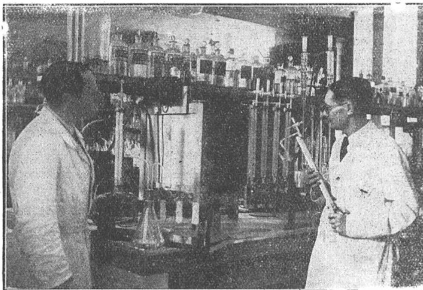
FIG. 5. — L'APPAREIL MANOMÉTRIQUE D'OTTO WARBURG POUR LA MESURE PRÉCISE DE FAIBLES VOLUMES GAZEUX
