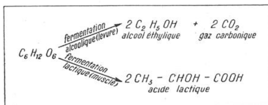
FIG. 3. — ÉQUATION DE PRINCIPE DE LA DÉGRADATION DES SUCRES PAR LA LEVURE ET DANS LE MUSCLE
