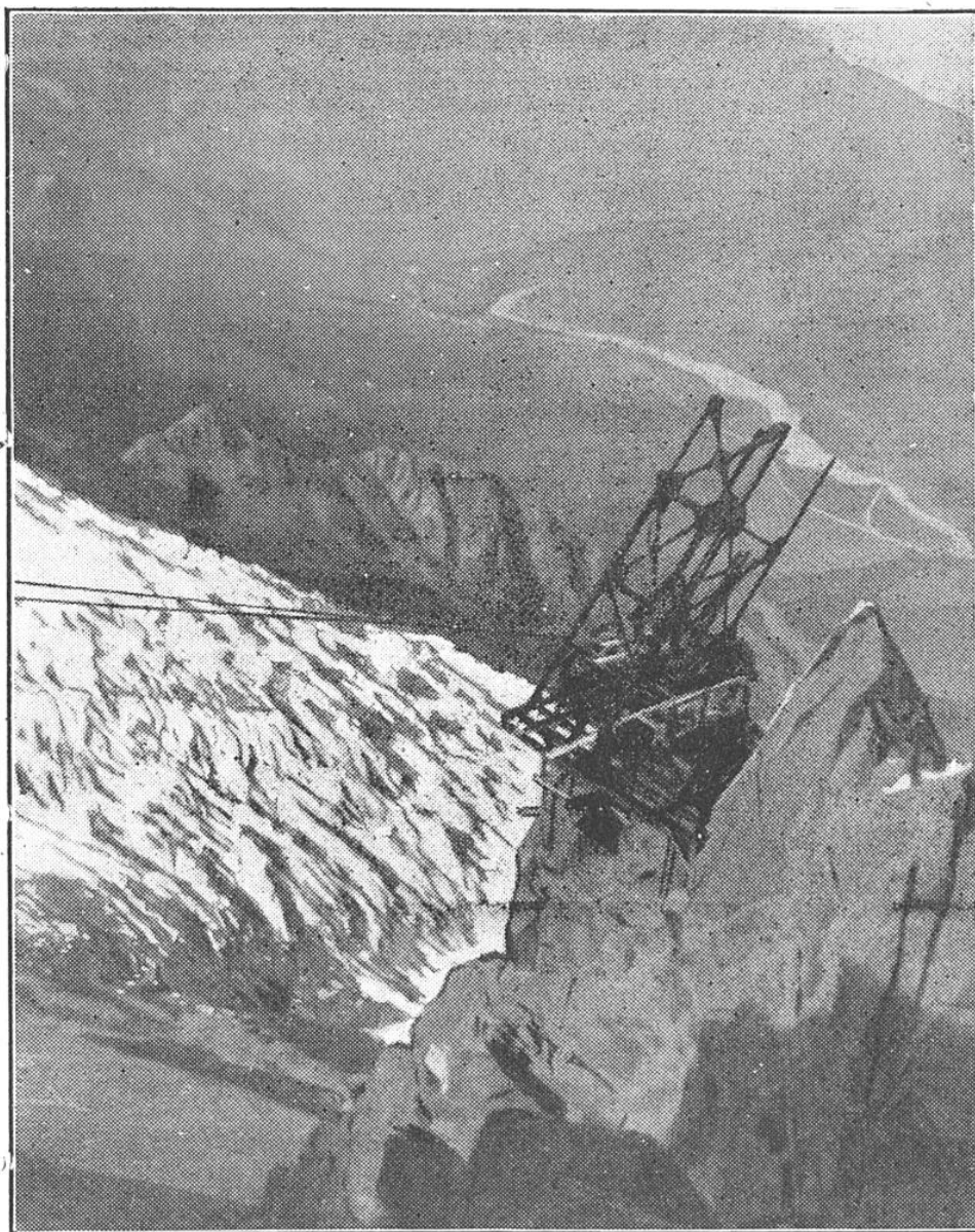
FIG. 2. — LE MONTAGE DU PYLONE DE L'ARÊTE (3 100 M D'ALTITUDE), AU-DESSUS DE LA VALLÉE DE CHAMONIX
