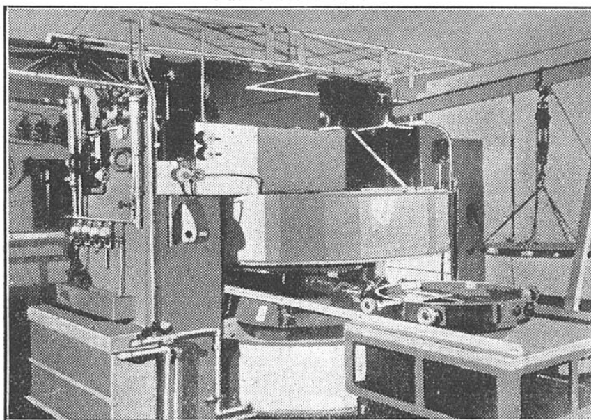
FIG. 1. — LE CYCLOTRON DE LA FONDATION DE RECHERCHES BIOCHIMIQUES DU FRANKLIN INSTITUTE DE PHILADELPHIE (ETATS-UNIS)
