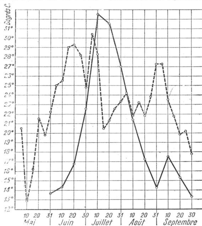
FIG. 5. — RAPPORT ENTRE LA MORBIDITÉ DE LA POLIOMYÉLITE ET LA TEMPÉRATURE AMBIANTE LORS DE L'ÉPIDÉMIE DE 1930 DANS LE BAS-RHIN (D'APRÈS LEVADITI, SCHMUTZ ET WILLEMIN)
