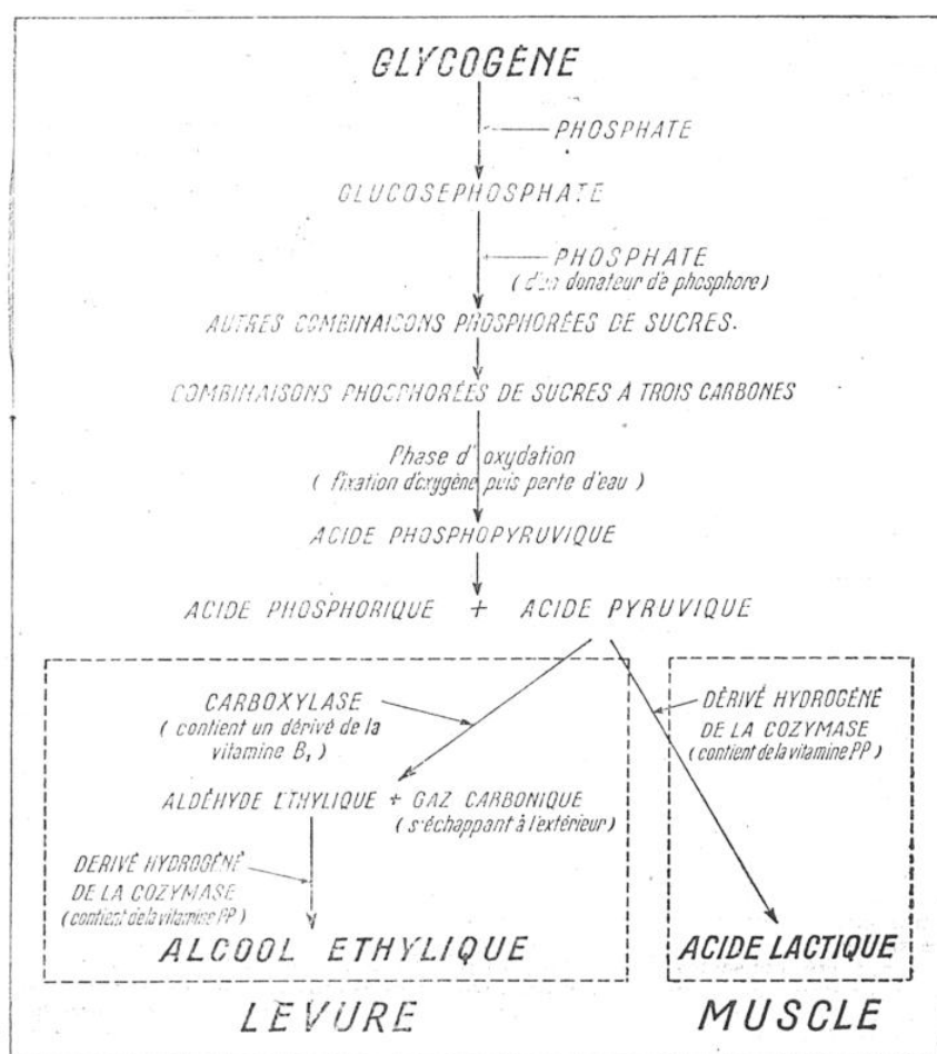
FIG. 4. — SCHÉMA TRÈS SIMPLIFIÉ DES ÉTAPES DE LA FERMENTATION ALCOLIQUE DE LA LEVURE ET DE LA FERMENTATION LACTIQUE DU MUSCLE
