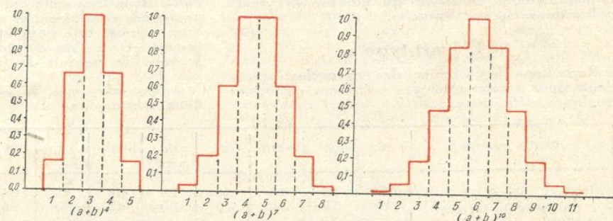
FIG. 8, 9 ET 10. — LES COEFFICIENTS DU BINOME
