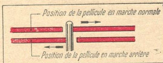
FIG. 8. — LA SUPERPOSITION CORRECTE DES IMAGES DANS LES DEUX SENS DE LA MARCHÉ NE PEUT ÊTRE ASSURÉE PAR SUITE DU JEU DES PERFORATIONS
