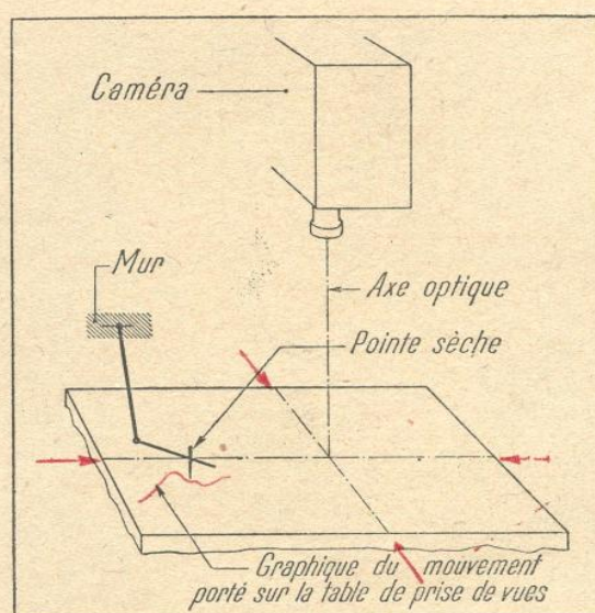
FIG. 11. — COMMENT ON RÈGLE LES MOUVEMENTS DE LA TABLE PORTANT LES DESSINS À ANIMER
