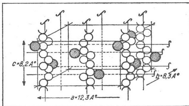
FIG. 7. — SCHÉMA DE LA CELLULE ÉLÉMENTAIRE DU CAOUTCHOUC. Ce serait une cellule orthorhombique (le système cristallin orthorhombique comporte trois axes de symétrie binaires; sa forme fondamentale est le prisme droit à base losange). L'axe c correspond à la direction de traction. La cellule contiendrait huit groupes isoprènes orientés parallèlement à cet axe et capables en outre de tourner autour de celui-ci. La densité calculée d'après ce modèle correspond bien à la densité réelle du caoutchouc, soit 0,92.
