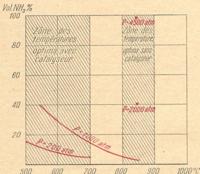
FIG. 5. — CONCENTRATIONS D'AMMONIAC RÉALISÉES À DIVERSES PRESSIONS ET TEMPÉRATURES
