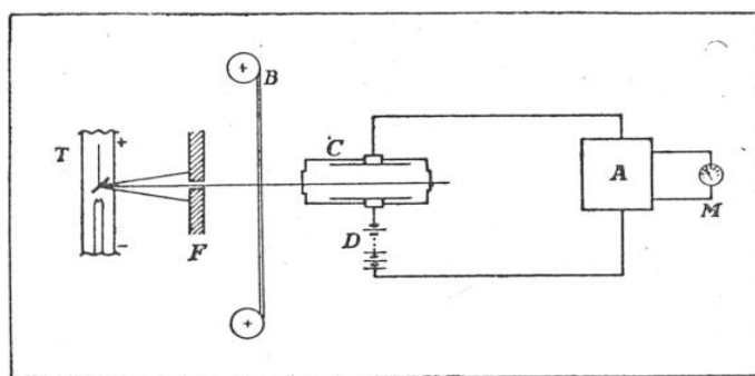
FIG. 9. — SCHÉMA DE LA MESURE DE L'HOMOGENÉITÉ D'UN CAOUTCHOU INDUSTRIEL
