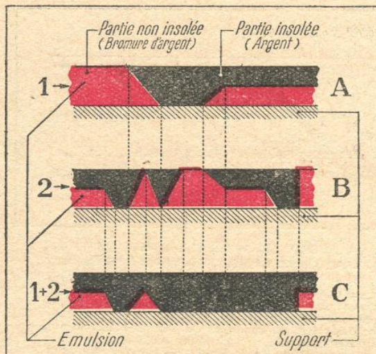
FIG. 6. — LE RÉSULTAT DE LA SUPERPOSITION DE DEUX IMAGES PHOTOGRAPHIQUES A DEMI-TEINTES.
