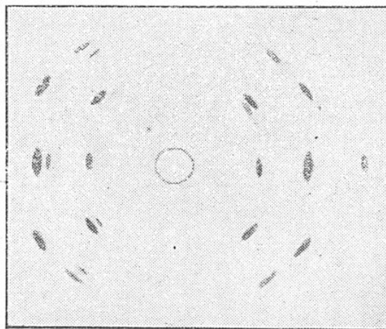
FIG. 4. — DIAGRAMME X DU CAOUTCHOUC ÉTIRÉ EN BANDE MINCE
