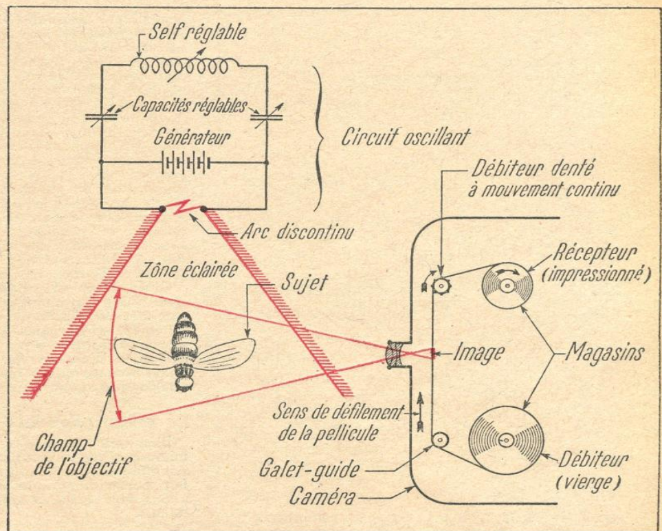
FIG. 2. — SCHÉMA DE PRINCIPE SIMPLIFIÉ D'UNE CAMÉRA POUR PRISES DE VUES ULTRARAPIDES
