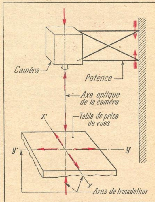
FIG. 9. — LES MOUVEMENTS QUE DOIT POUVOIR EFFECTUER LE MATÉRIEL DE PRISE DE VUES POUR L'ANIMATION DES DESSINS
