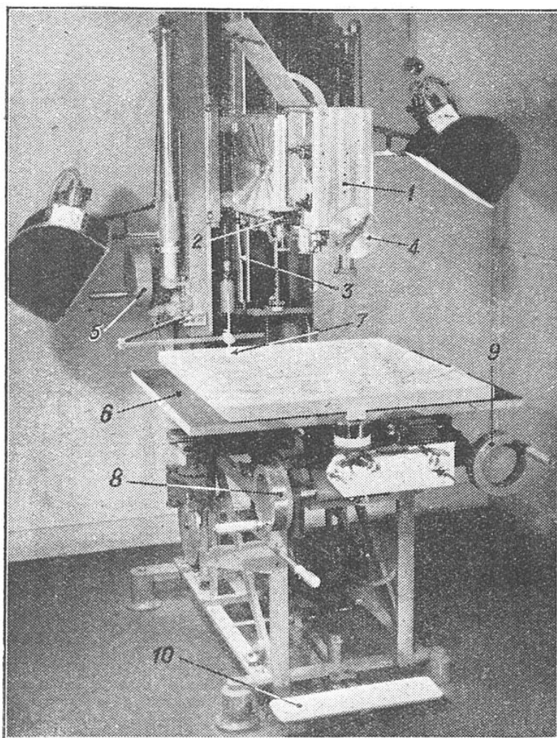
FIG. 12. — CAMÉRA SPÉCIALISÉE ET TABLE DE PRISE DE VUES SPÉCIALEMENT CONÇUE POUR LES FILMS SCIENTIFIQUES
