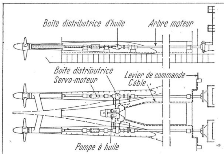
FIG. 2. — SCHÉMA DE PRINCIPE DE LA COMMANDE DE L'HÉLICE A PAS VARIABLE KAMOWA (GÖTAVERKEN)
