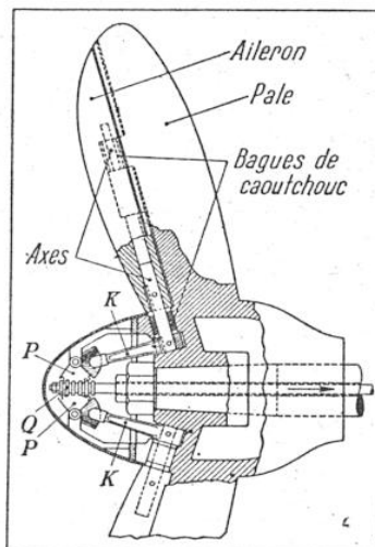
FIG. 3. — SCHÉMA DE L'HÉLICE STONE. K, BIELLETTES; P, SECTEUR DENTÉ; Q, CRÉMAILLÈRE.
