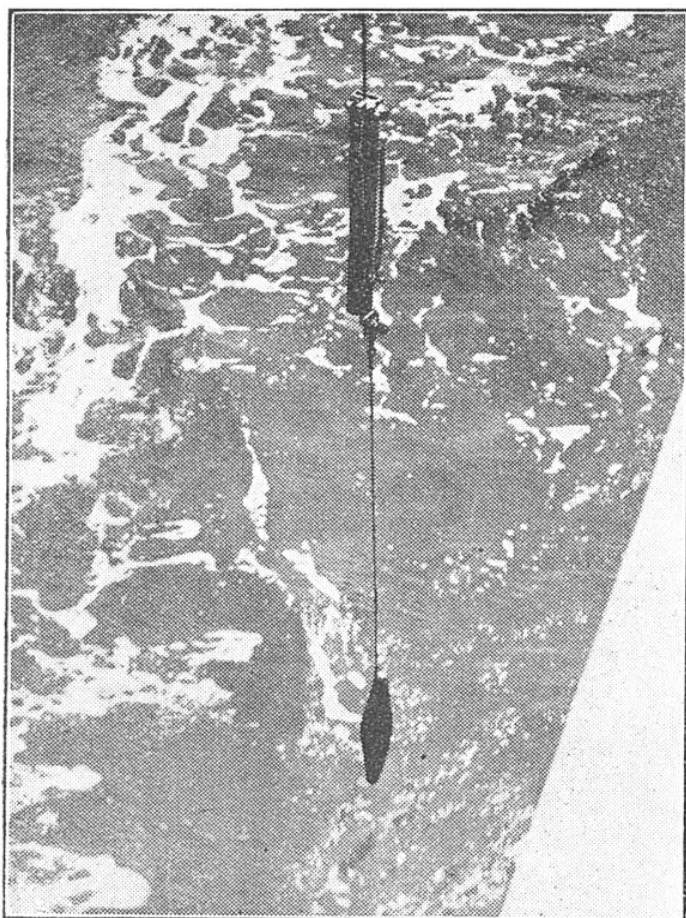
FIG. 4. — MISE A L'EAU D'UNE EOUTEILLE DE PRISE D'EAU AUTOMATIQUE POUR LE PRÉLÈVEMENT D'ÉCHANTILLONS D'EAU A DIVERSES PROFONDEURS
