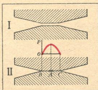
FIG. 2. — DISPOSITIF POUR L'OBTENTION DE PRESSIONS DE L'ORDRE DE 300 000 KG/CM 2
