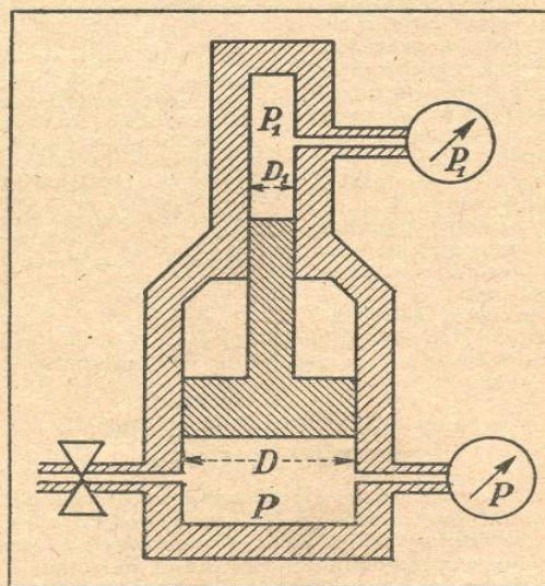
FIG. 3. — TARAGE DES MANOMÈTRES A ULTRAPRESSIONS
