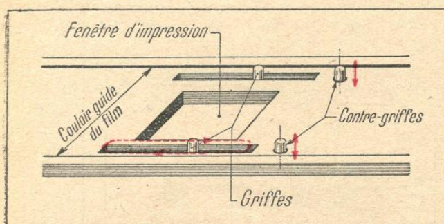
FIG. 7. — SCHÉMA DU SYSTÈME D'ENTRAÎNEMENT ET D'IMMOBILISATION DE LA PELLICULE DANS UNE CAMÉRA
