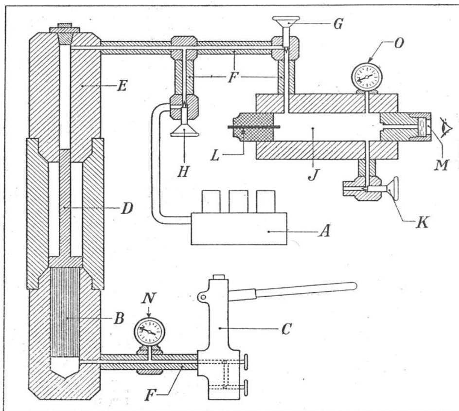
FIG. 1. — SCHÉMA D'UN COMPRESSEUR DE GAZ POUR 25\,000\text{ kg/cm}^2
