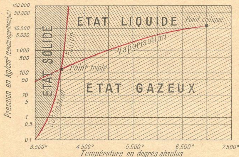
FIG. 4. — DIAGRAMME DES ÉTATS DU CARBONE (D'APRÈS BASSET)
