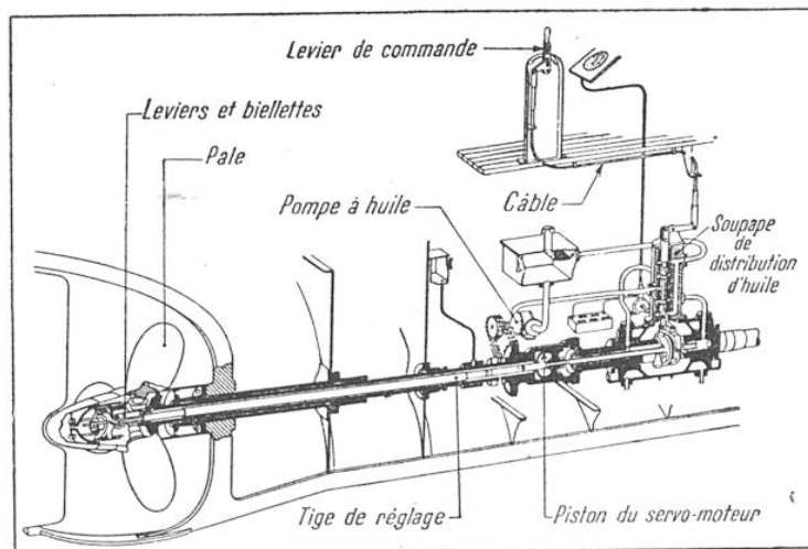
FIG. 1. — SCHÉMA DE PRINCIPE DE LA COMMANDE DE L'HÉLICE A PAS VARIABLE ESCHER WYSS
