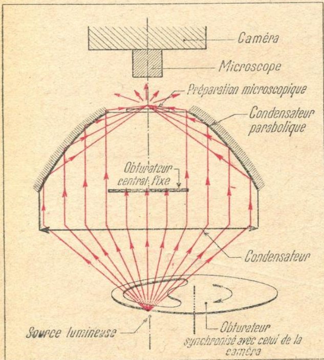
FIG. 3. — UN DES MONTAGES OPTIQUES PERMETTANT L'ÉCLAIRAGE LATÉRAL DES PRÉPARATIONS POUR L'ULTRAMICROSCOPIE
