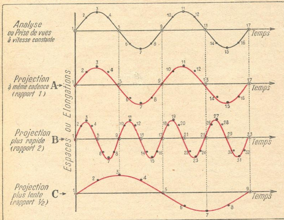
FIG. 1. — LE PRINCIPE DE L'ACCÉLÉRATION ET DU RALENTISSEMENT D'UN MOUVEMENT CINÉMATOGRAPHIÉ
