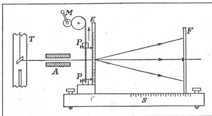
FIG. 2. — SCHÉMA D'UN SPECTROGRAPHE A ÉTIREMENT POUR L'ÉTUDE DU CAOUTCHOUC
