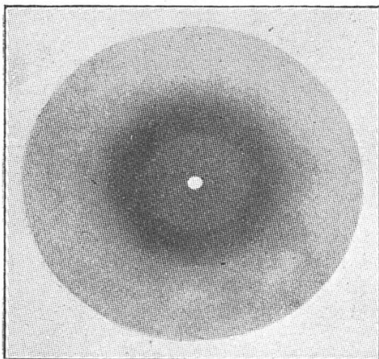
FIG. 3. — DIAGRAMME X DU CAOUTCHOUC NON ÉTIRÉ
