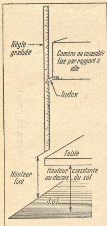
FIG. 10. — COMMENT ON REPÈRE LA POSITION DE LA CAMÉRA POUR LES SURIMPRESSIONS
